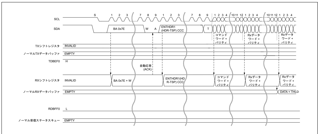
図 33.56 HDR データ書き込み転送 (HDR-TSP、TSL) タイミング (1/2)
