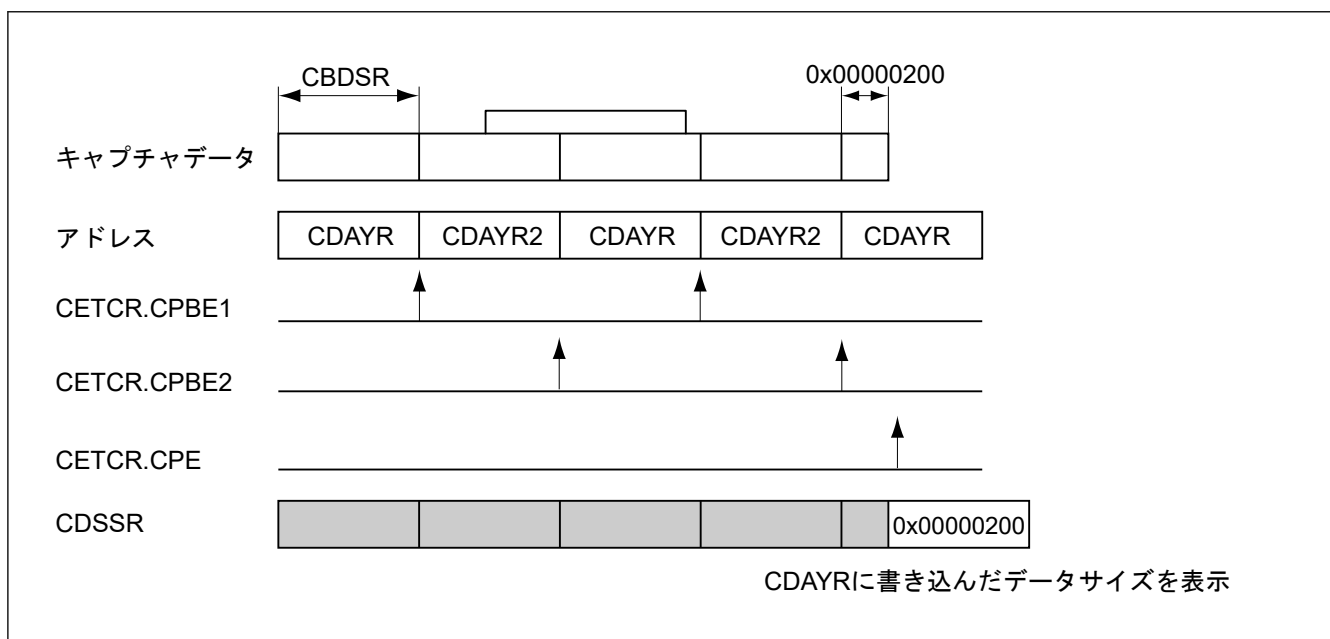
図 53.49 バンドル書き込み時の CDSSR 動作タイミングイメージ図 (バンドル書き込み終了とキャプチャ終了が異なる場合)
