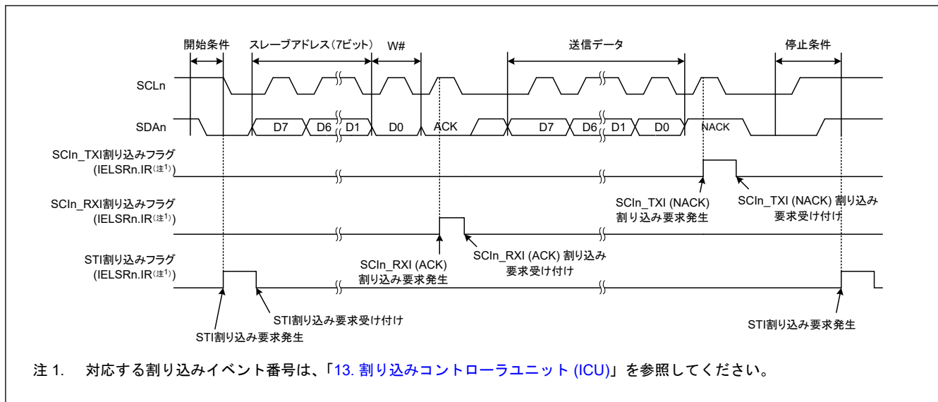
図 31.92 簡易 IIC モードにおけるマスタ送信の動作例 2 (7 ビットスレーブアドレス、ACK 割り込み、NACK 割り込み使用時) (ICR.IICINTM = 0)
