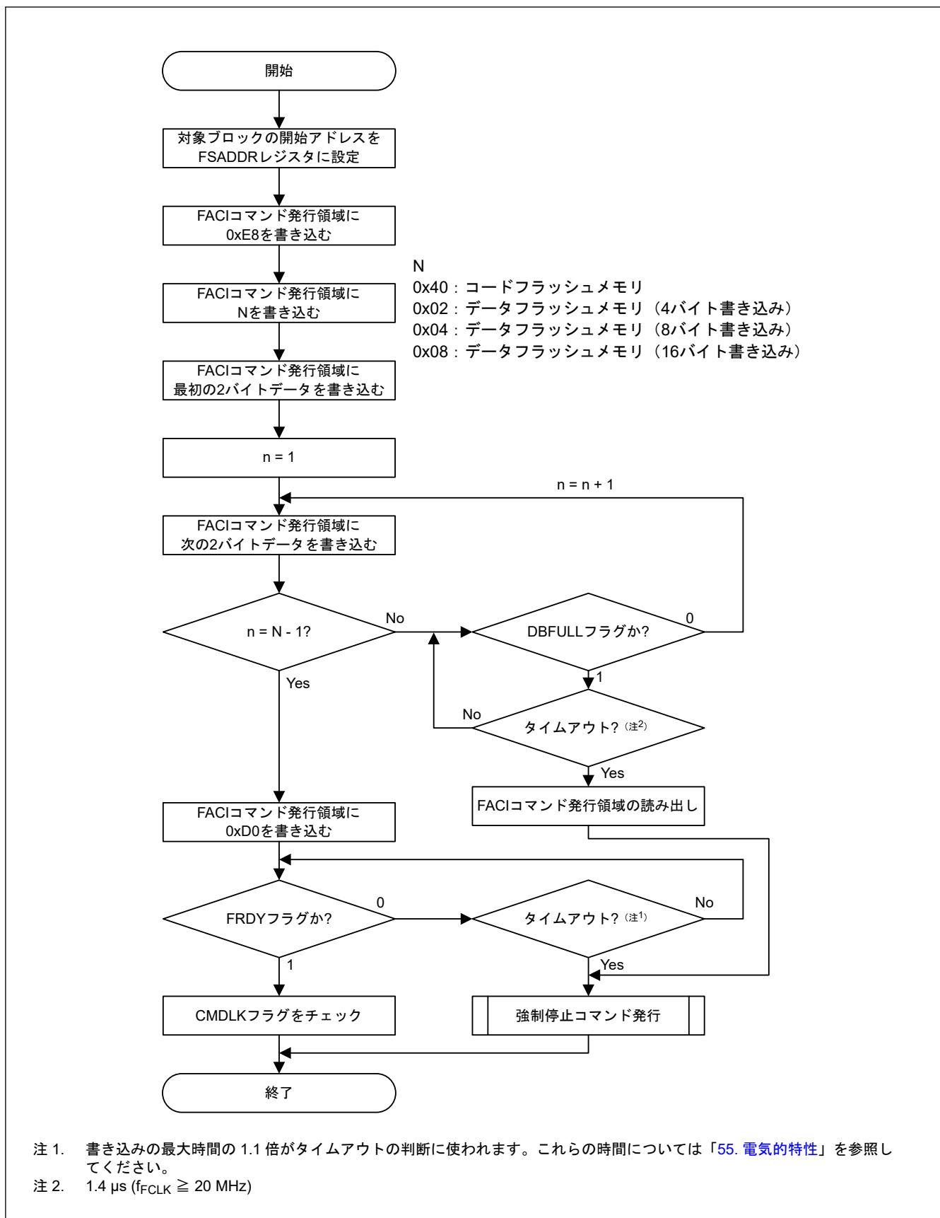
図 52.14 プログラムコマンドの使用フロー
