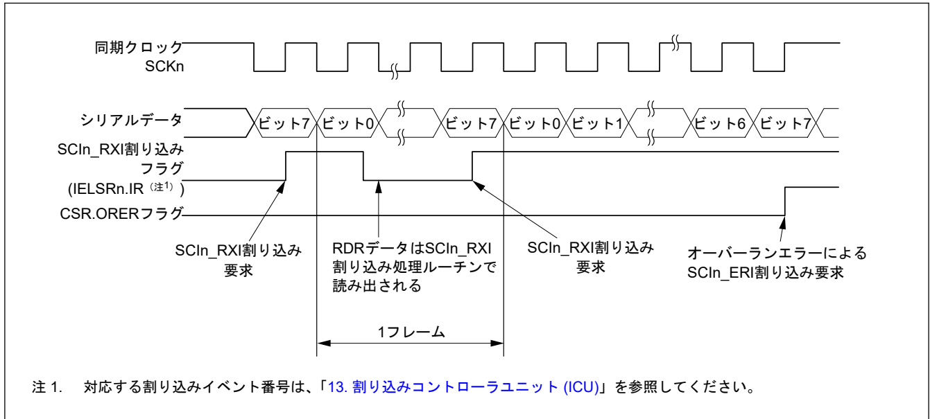
図 31.67 クロック同期式モードにおけるシリアル受信の動作例 (1) (RTS 機能を使用しない場合)
