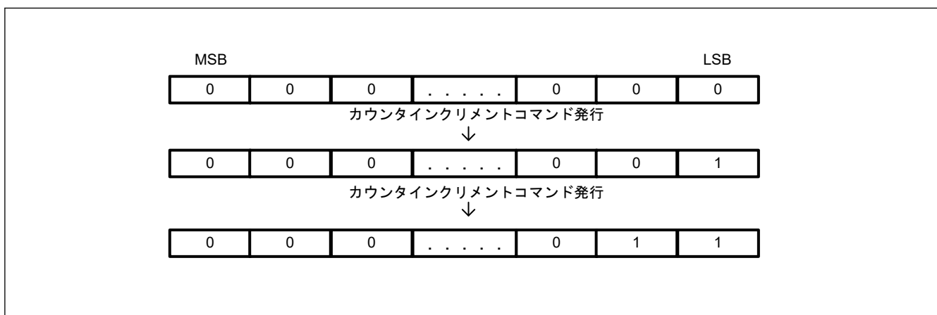
図 52.43 アンチロールバックカウンタのインクリメントのイメージ
