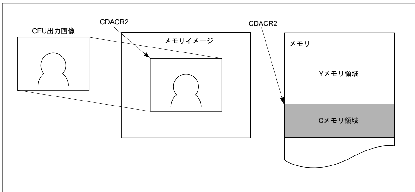
図 53.51 キャプチャ画像と色差成分メモリ領域の関係
