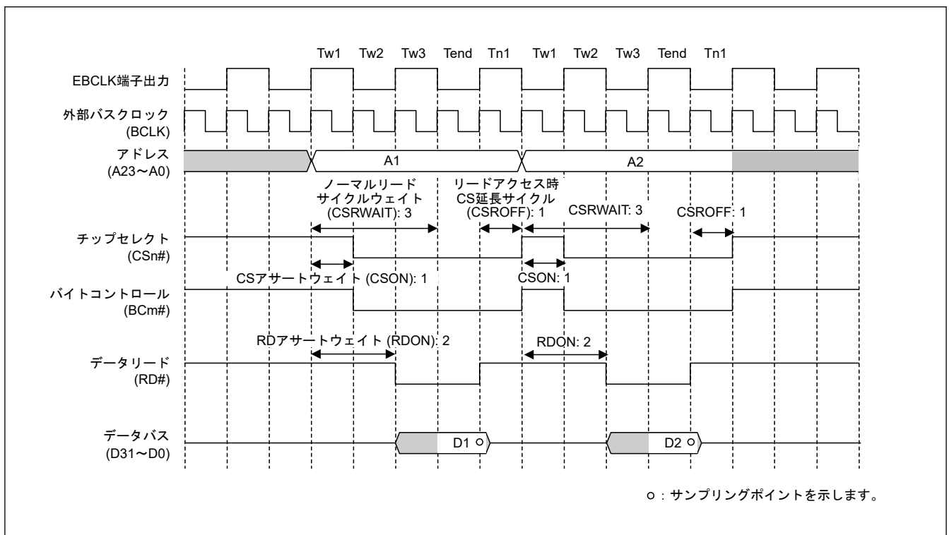
図 14.13 ノーマルリードアクセスの動作例 (EBCLK 端子出力選択ビットで BCLK の 2 分周を設定した場合、および 1 転送要求に対して 2 回バスアクセスが発生する場合) (n = 0~7, m = 0~3)
