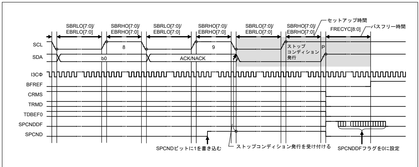
図 33.81 ストップコンディション発行タイミング (SPCND ビット)
