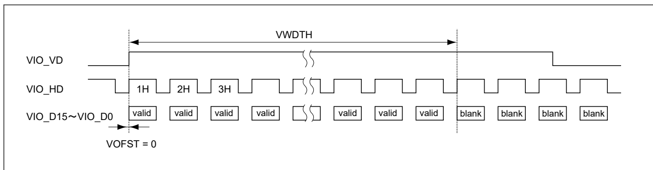
図 53.21 垂直キャプチャタイミング
