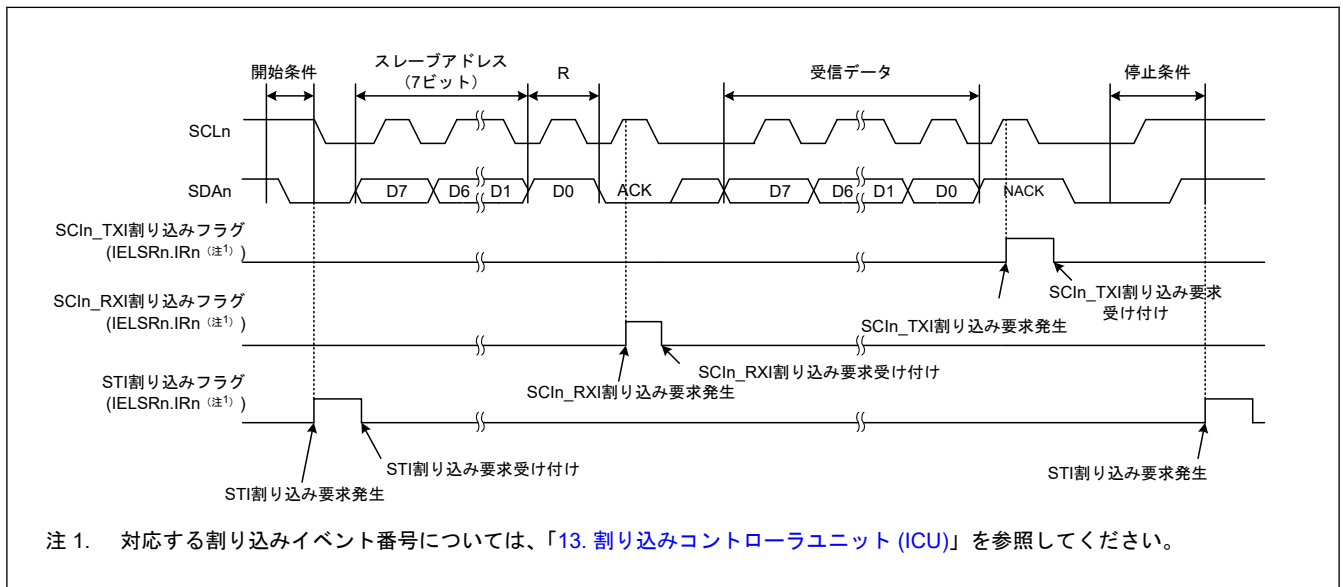
図 31.95 簡易 IIC モードにおけるマスタ受信の動作例 (7 ビットスレーブアドレス、ACK 割り込み、NACK 割り込み使用時) (ICR.IICINTM = 0)
