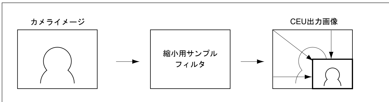
図 53.32 キャプチャ画像の縮小
