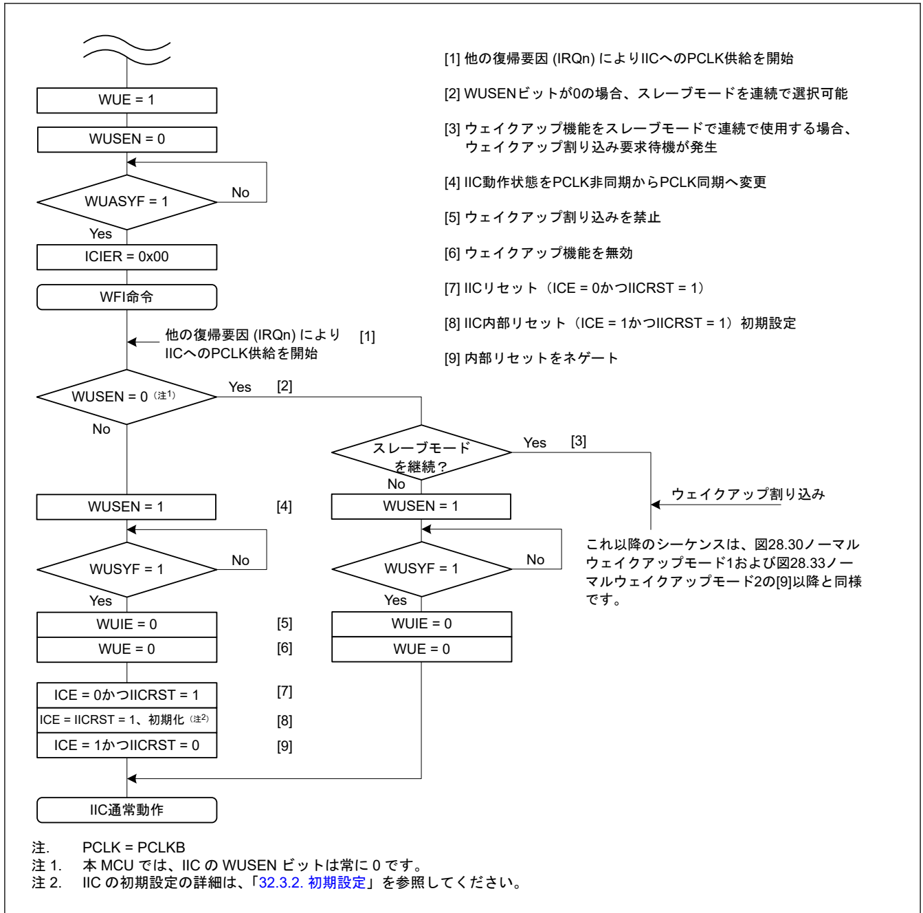
図 32.31 ノーマルウェイクアップモード 1 および 2 の動作例 (IIC ウェイクアップ割り込み以外の割り込み (たとえば IRQn) によるウェイクアップの場合)
