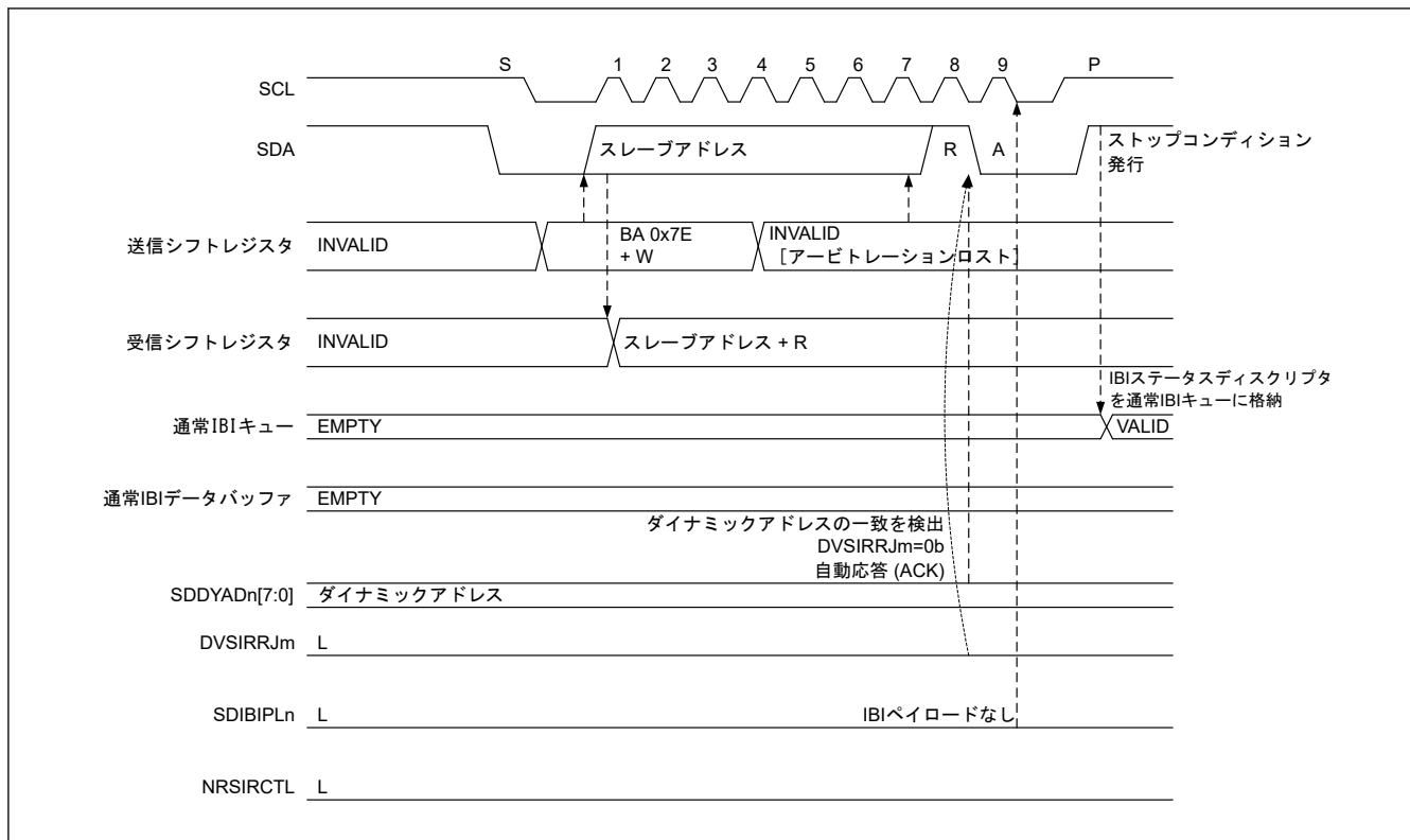
図 33.101 スレーブ割り込み要求 : ACK かつ DVIBIPL が 0 の場合
