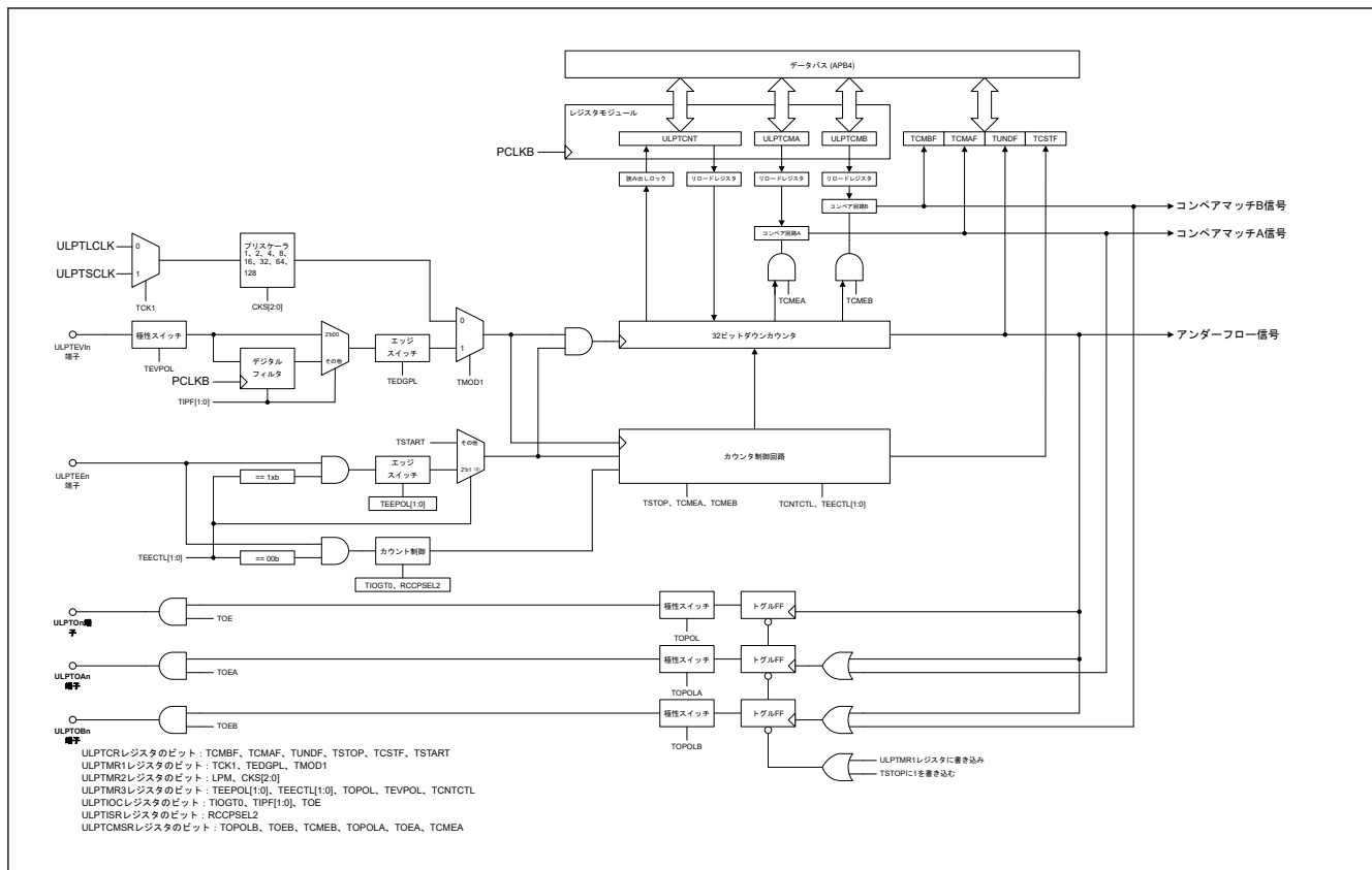
図 23.1 ULPT のブロック図
