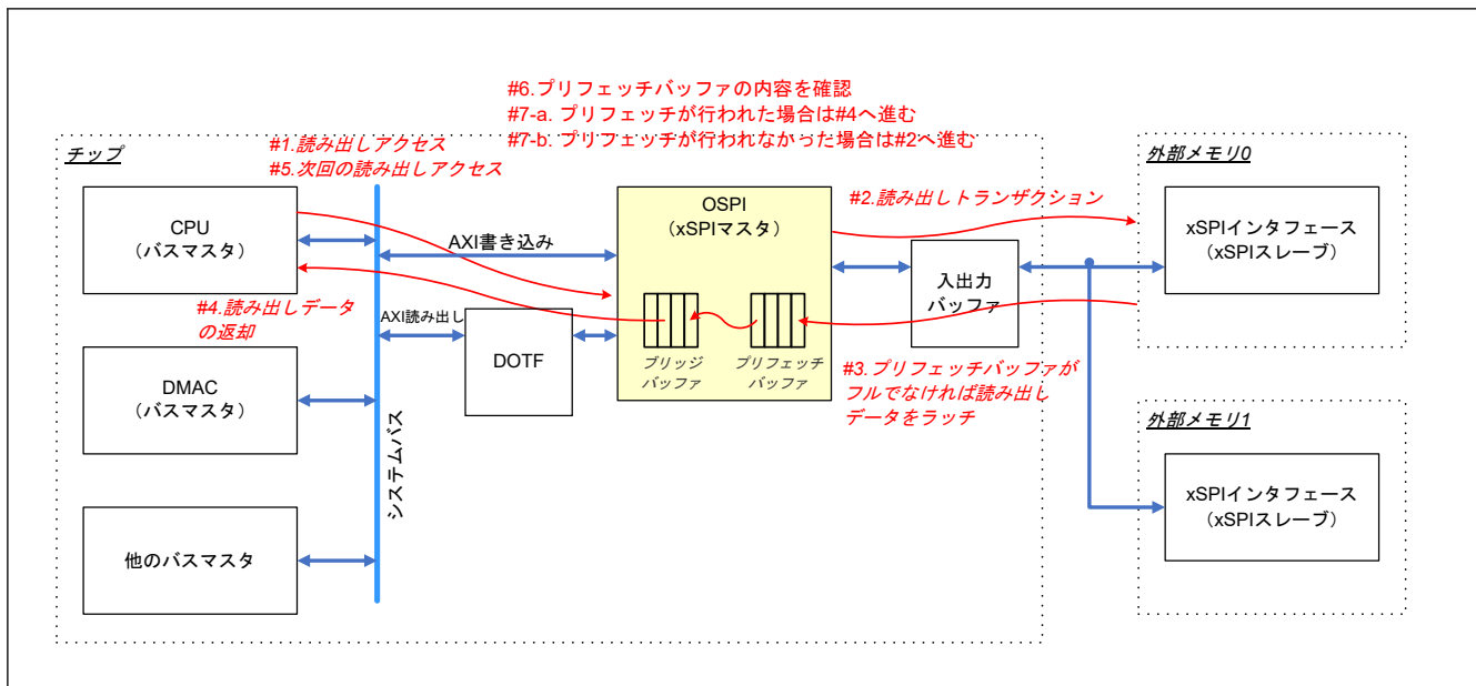
図 37.18 プリフェッチ許可時のメモリ領域の読み出しアクセス
