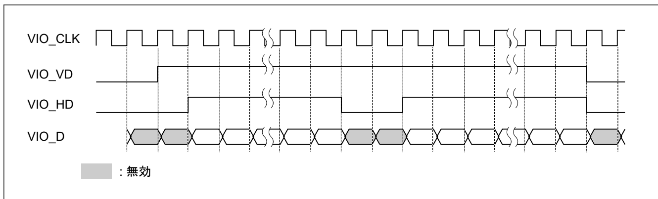
図 53.12 データイネーブル取り込みタイミング (VD が High の期間内に HD がアサート (High))
