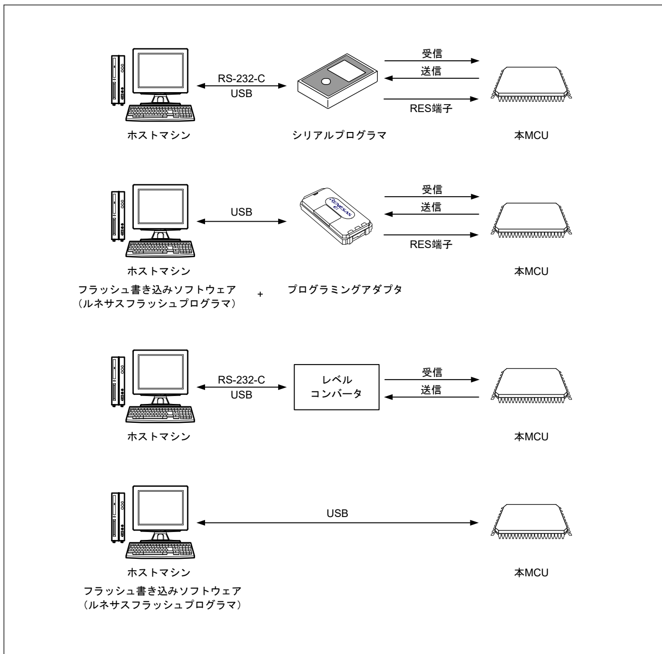
図 52.49 フラッシュメモリを書き換えるための環境
