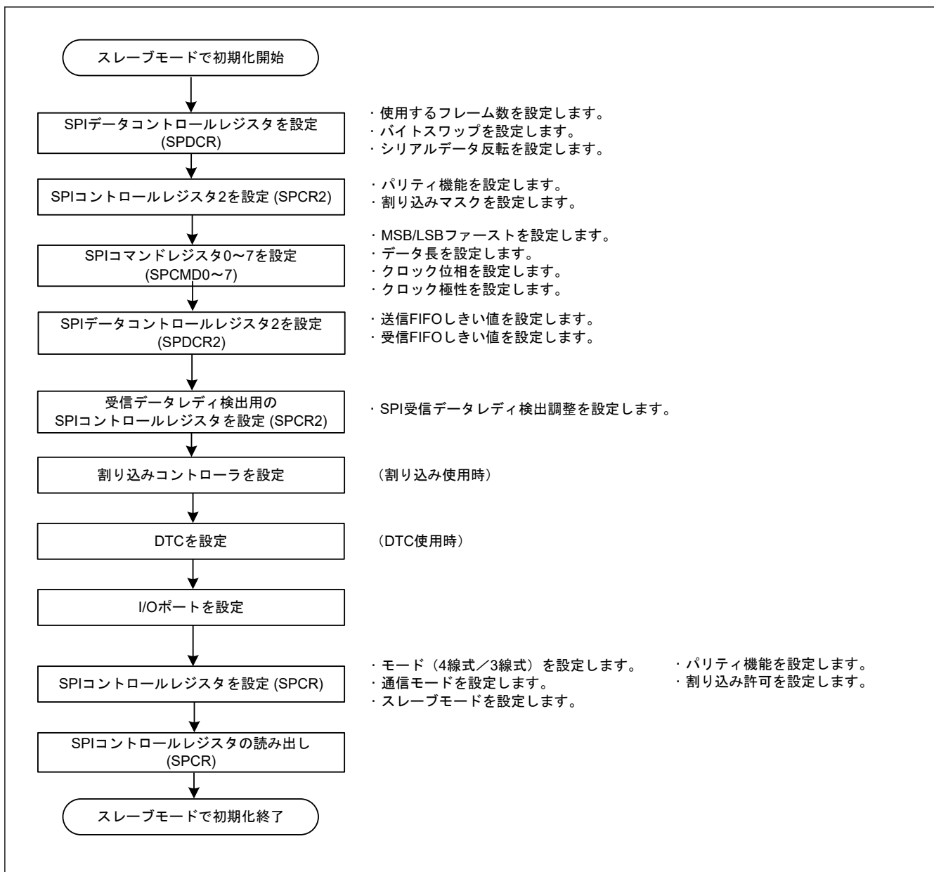
図 36.77 スレーブモード時のクロック同期式動作の初期化フロー例
