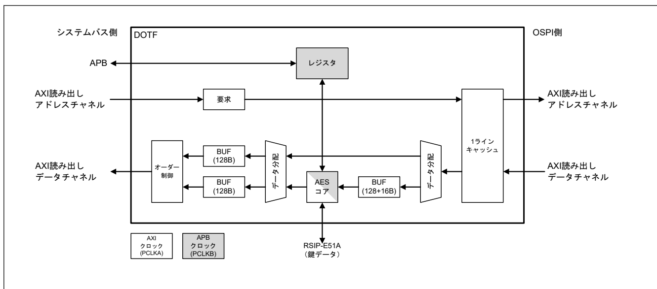
図 38.1 ブロック図
