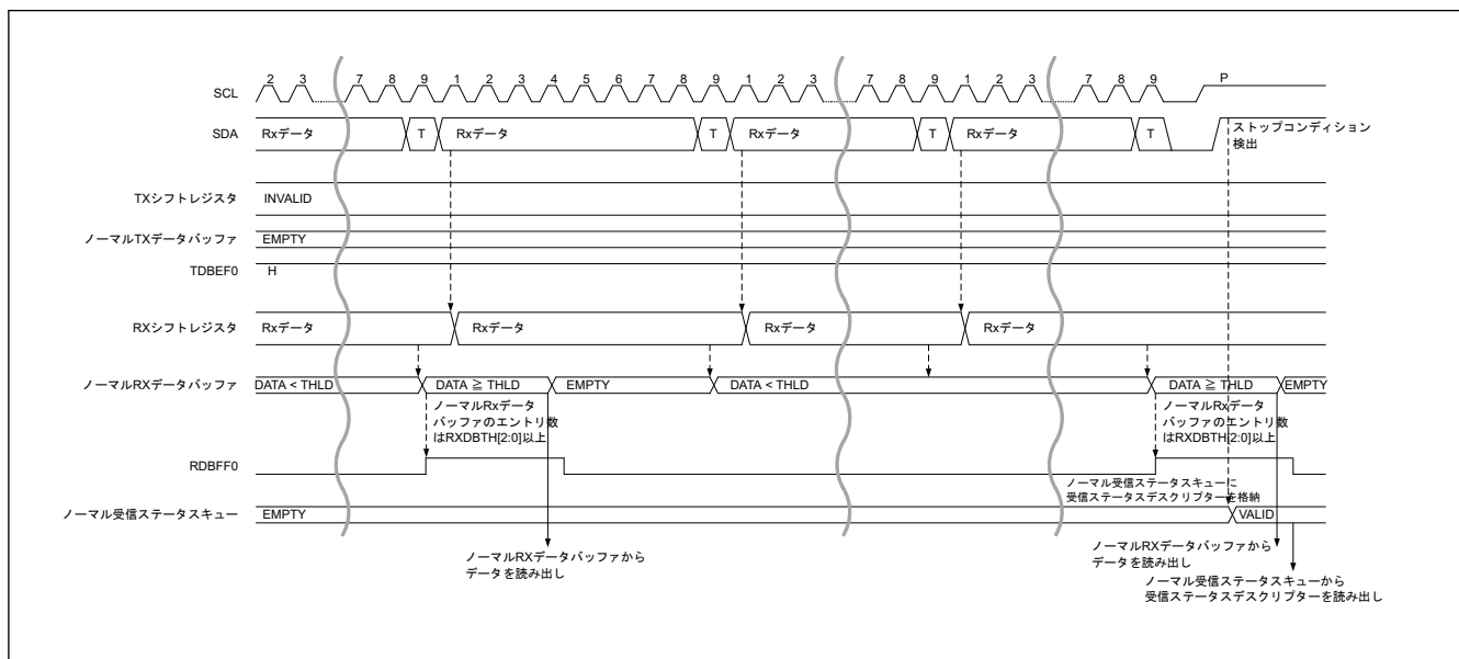
図 33.46 SDR データ書き込み転送タイミング (2/2)
