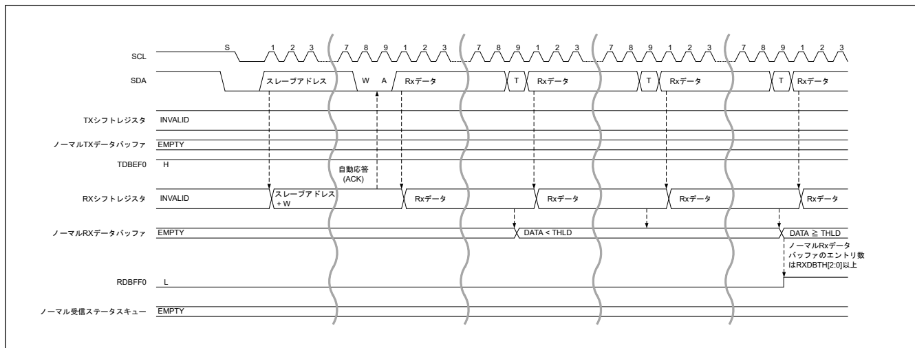
図 33.45 SDR データ書き込み転送タイミング (1/2)
