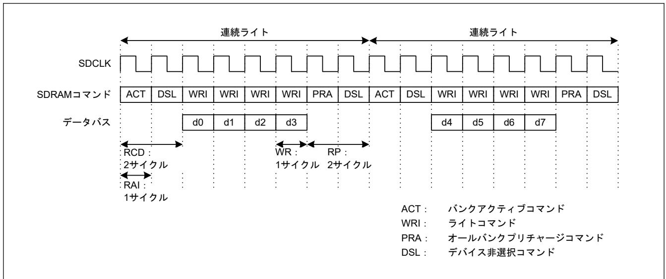
図 14.66 連続ライトタイミング例 (2)
