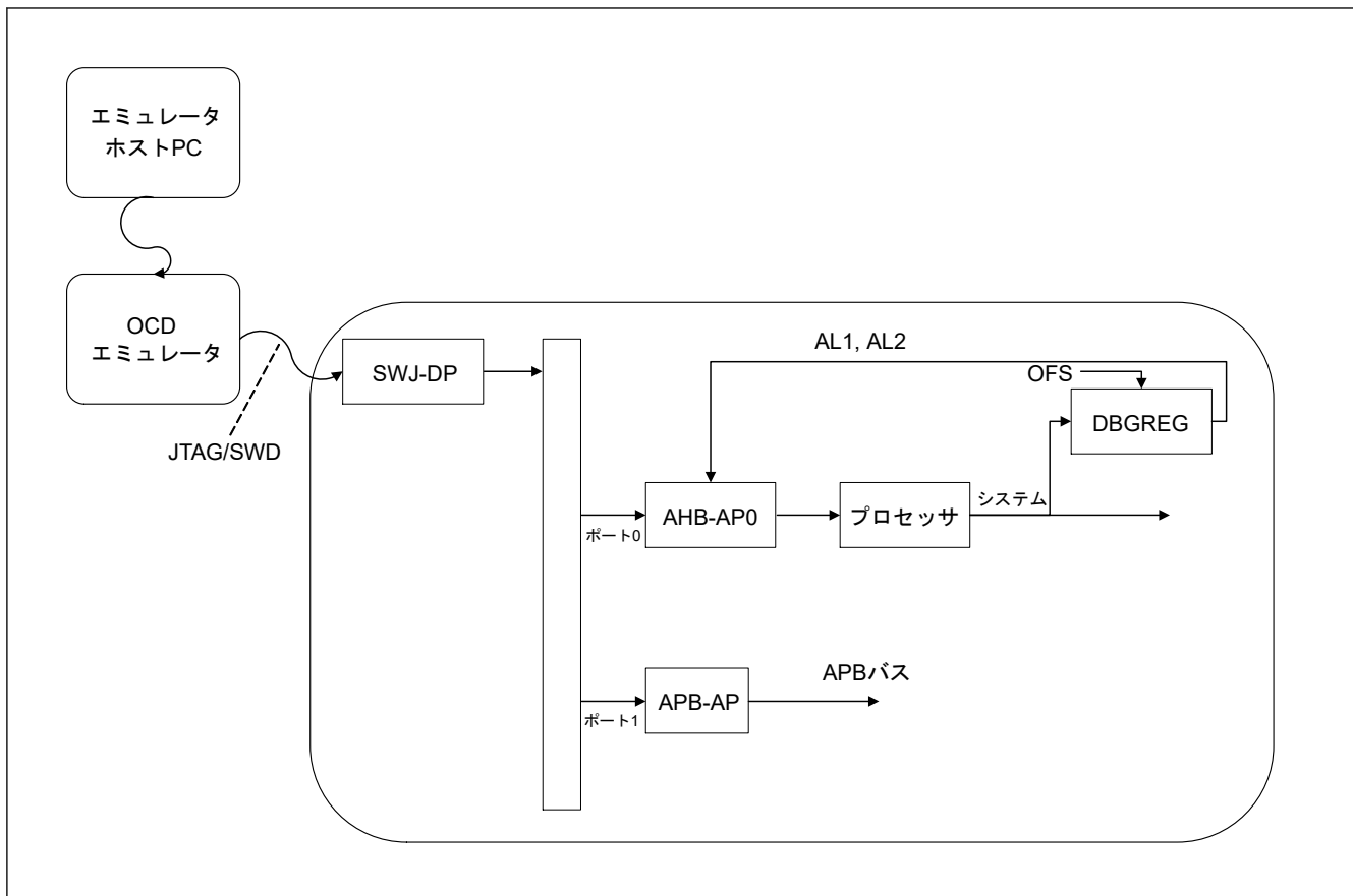
図 2.6 ソフトウェアを使用した認証レベルの制御
