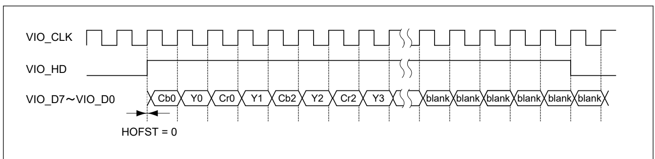
図 53.20 HD がデータイネーブル信号の場合のタイミング (8 ビットインタフェース)
