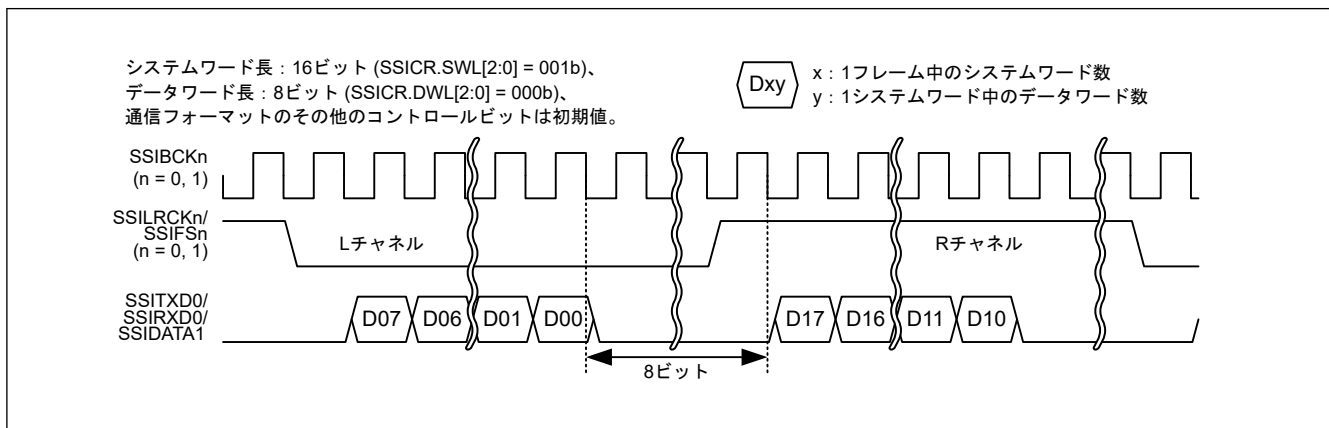
図 39.36 パディングビット転送の例 (I 2 S フォーマット、システムワード長 > データワード長)
