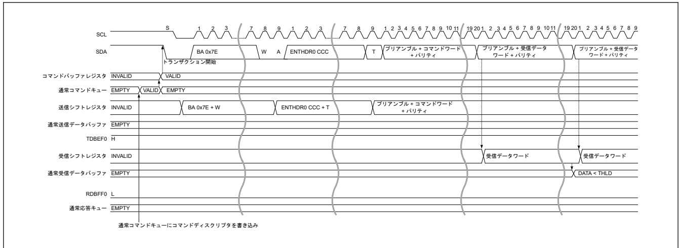
図 33.30 HDR データ読み出し転送 (HDR-DDR) タイミング (1/2)
