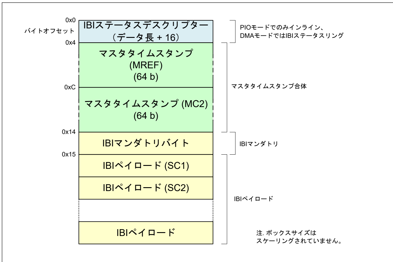
図 33.110 IBI イベント用のマスタタイムスタンプカウンタ
