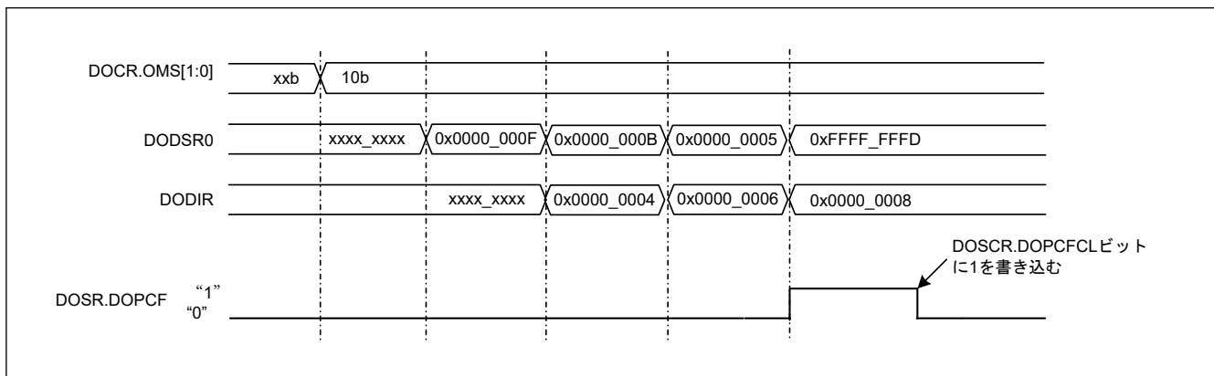
図 49.9 データ減算モードの動作例
