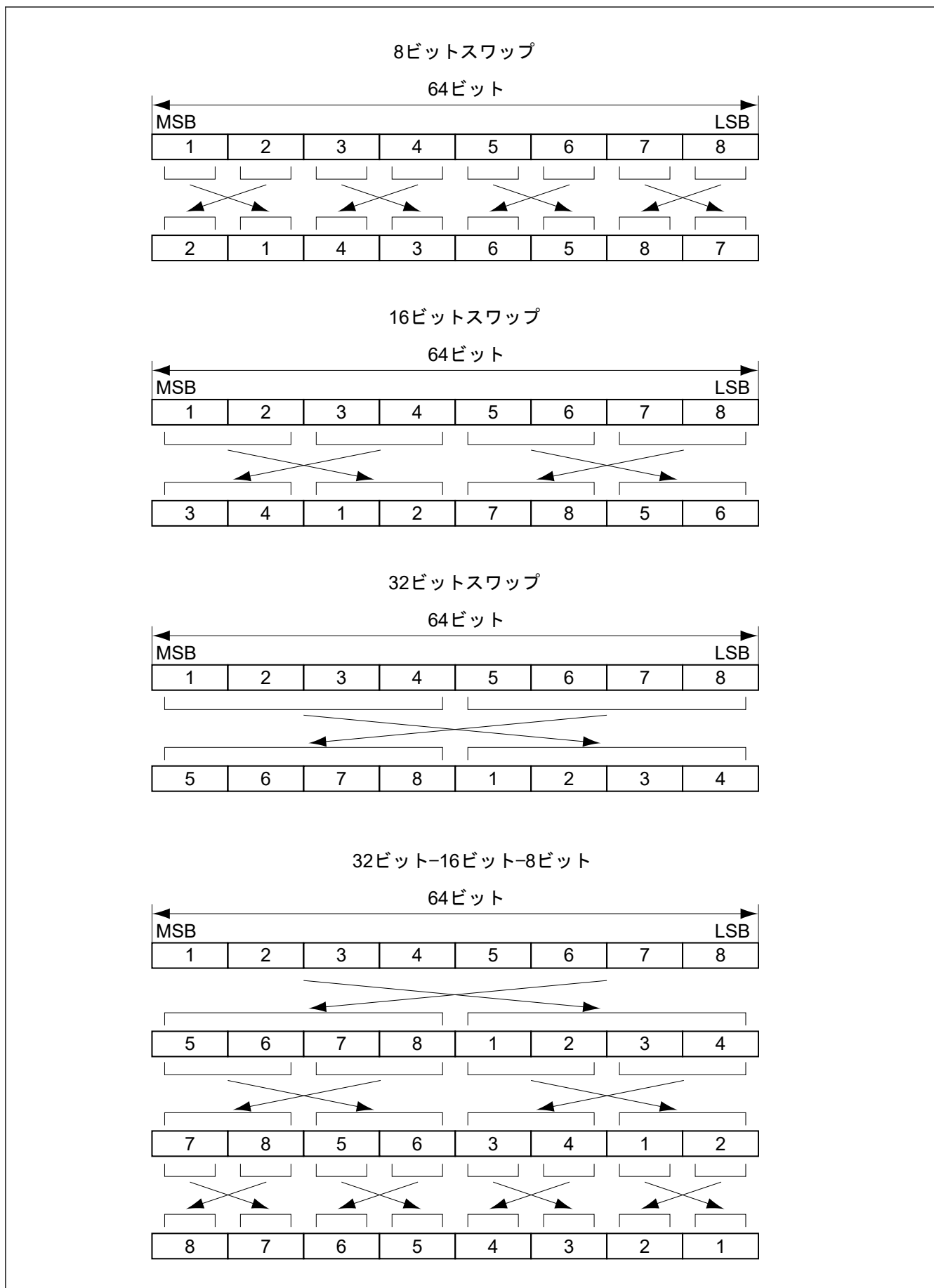
図 53.44 データライナーによるデータ入れ替え
