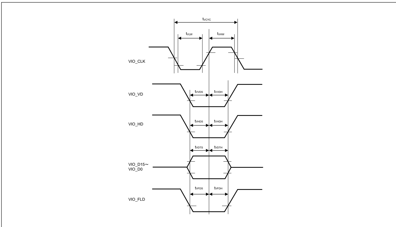
図 55.101 VIO_CLK の立ち上がりエッジによるデータキャプチャのキャプチャエンジンユニットモジュール信号タイミング
