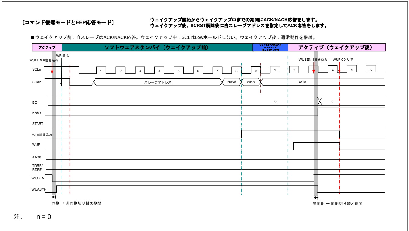
図 32.37 コマンドリカバリモードとEEP 応答モードのタイミング
