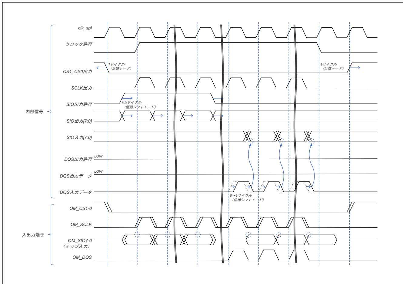
図 37.9 OM_DQS あり SDR のタイミング制御
