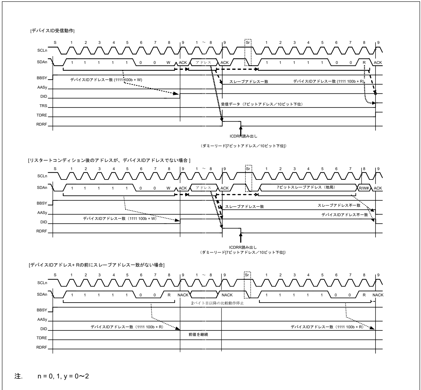
図 32.28 デバイス ID 受信時の AASn、DID フラグのセット/クリアタイミング
