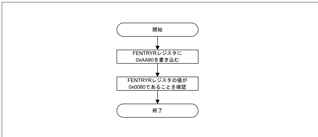
図 52.11 データフラッシュ P/E モードへの遷移手順
