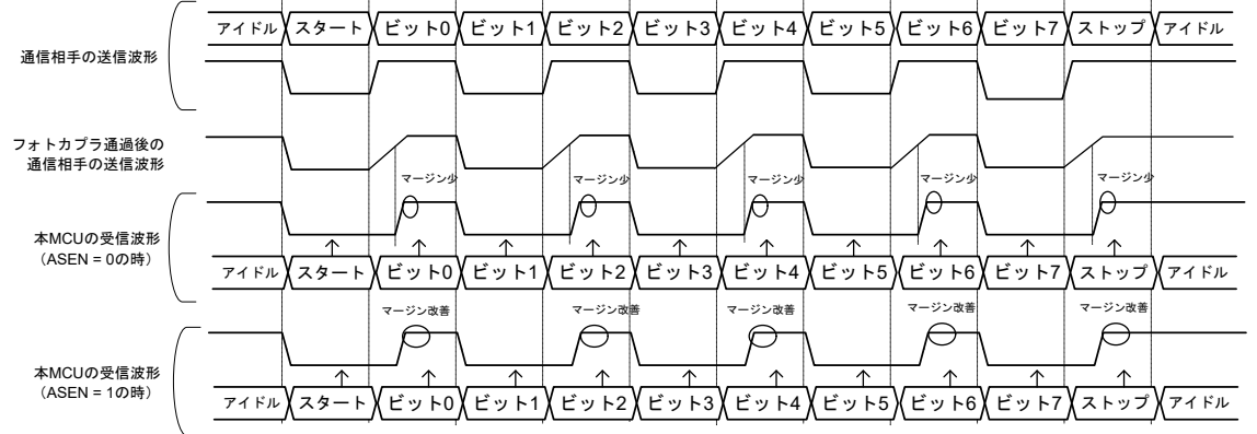
図 31.28 受信サンプリングタイミング調整機能による受信マージン向上の例
