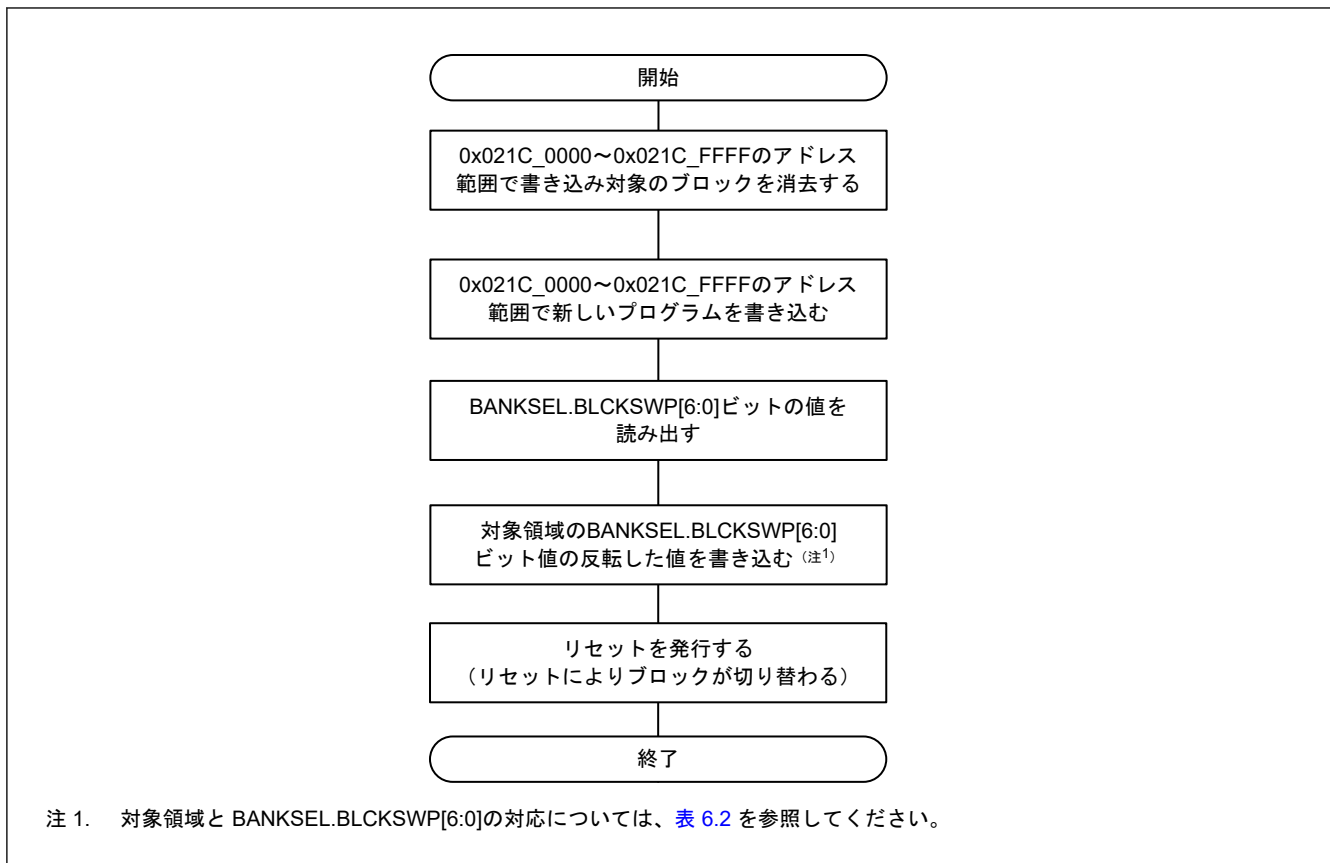
図 52.36 セキュアエアリアスのブロックスワップ選択フロー例 (2 MB のコードフラッシュメモリを持つ製品の場合)
