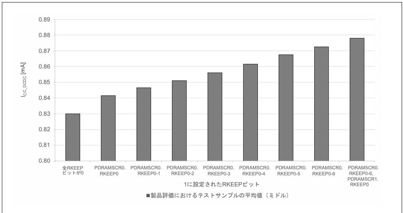
図 55.8 1 SRAM ステートあたりのソフトウェアスタンバイ電流 (参考データ)
