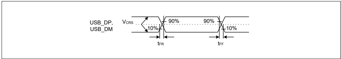
図 55.106 フルスピードモードにおける USB_DP、USB_DM の出カタイミング
