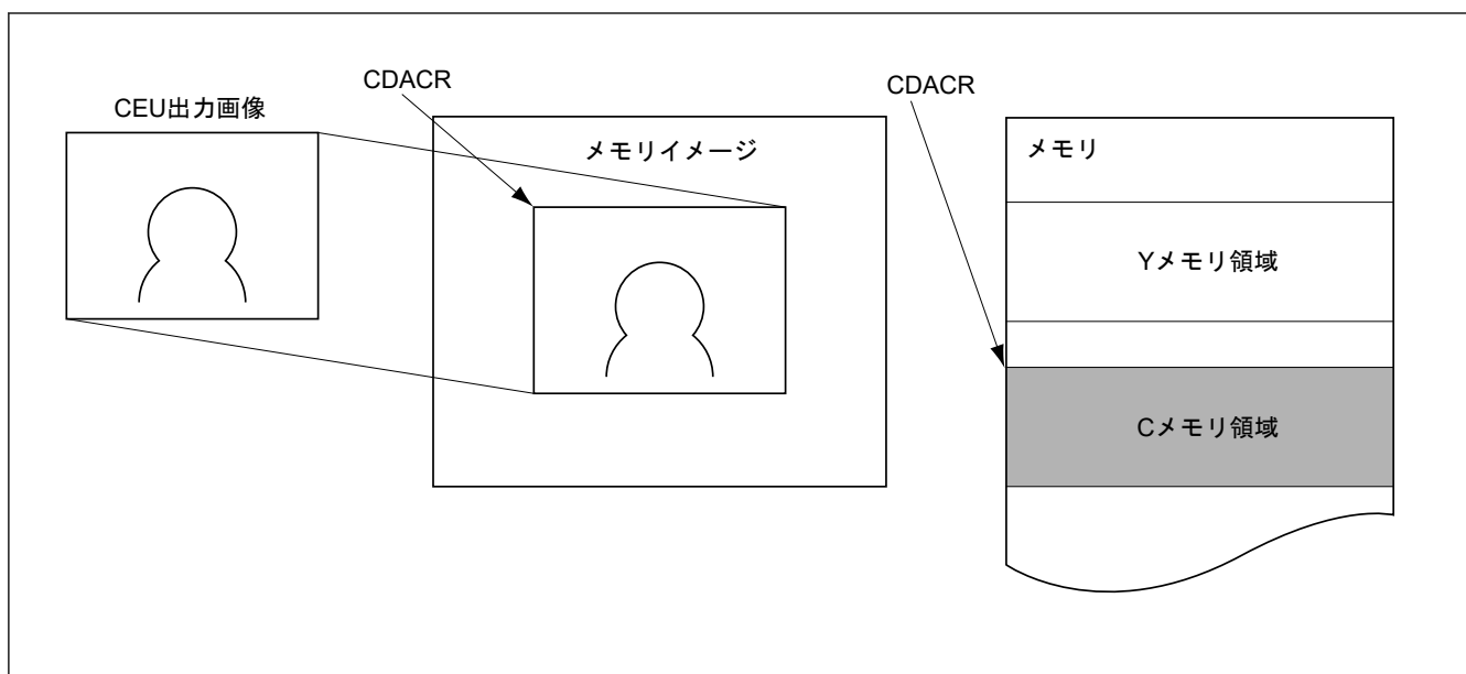
図 53.35 キャプチャ画像と色差成分メモリ領域の関係
