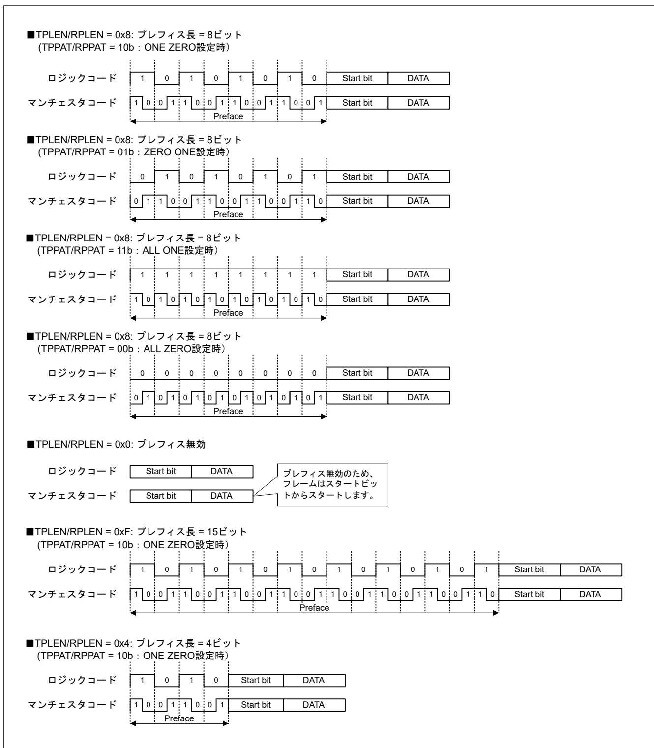
図 31.47 プレフィスパターンの設定例
