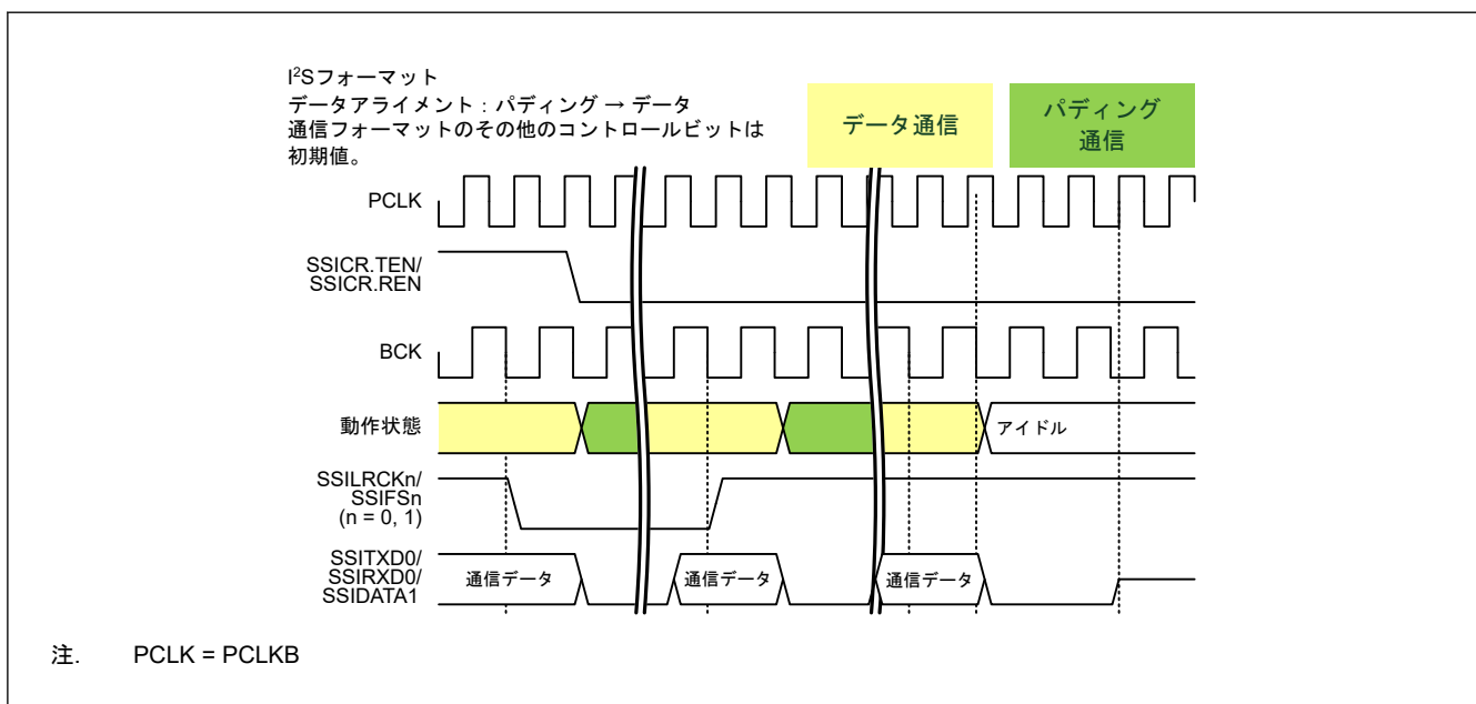
図 39.50 データ通信からの停止（パディングビットあり）
