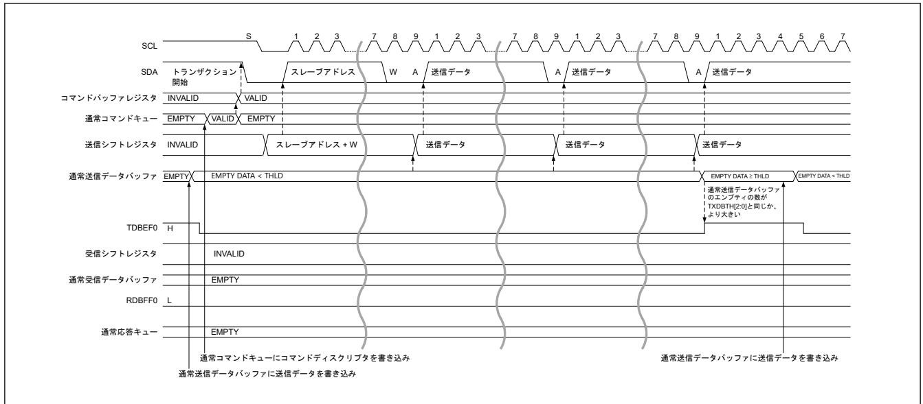
図 33.18 レガシー I 2 C メッセージデータ書き込みタイミング (1/2)
