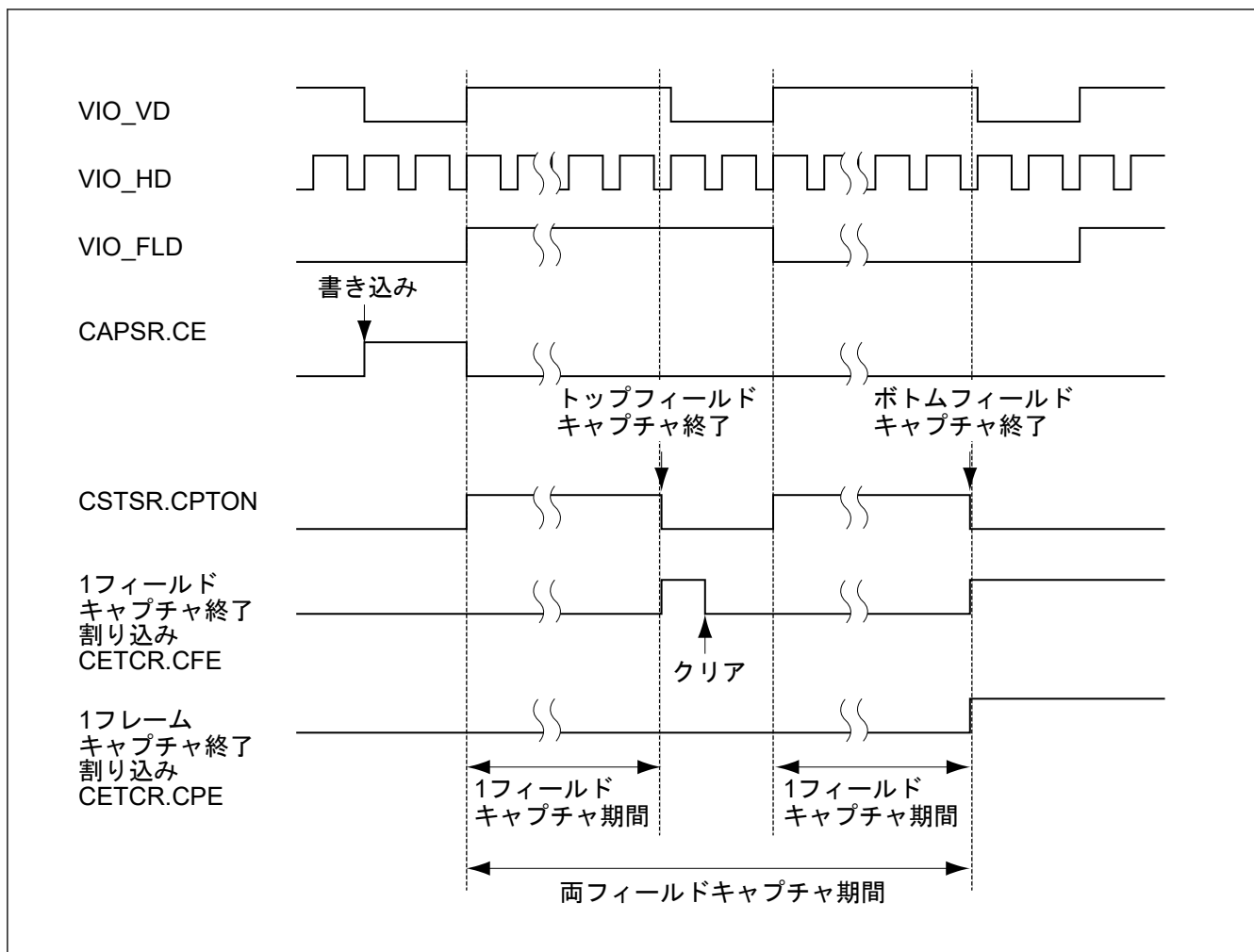
図 53.23 両フィールド画像キャプチャの1フレームキャプチャ終了割り込みおよび1フィールドキャプチャ終了割り込み
