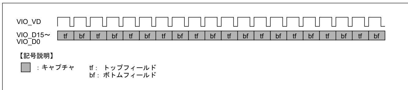
図 53.26 インターレース入力方式での両フィールド連続キャプチャ（起動直後の画像がトップフィールドの場合 (FCI[1:0] = 00b)
