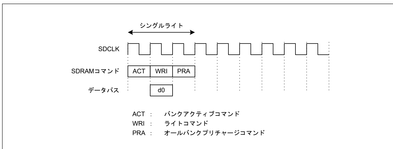
図 14.45 シングルライトのタイミング例 (最短のタイミングを設定したとき)
