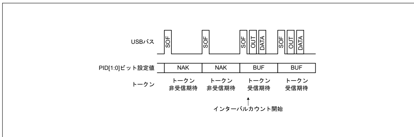
図 30.14 IITV[2:0] = 0 の場合のフレームとトークン受信期待の関係
