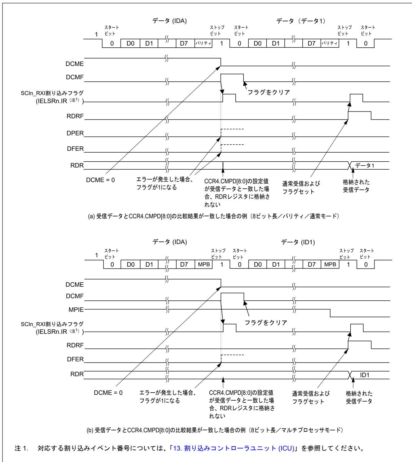
図 31.9 アドレス一致検出の例 (1) (通常モードとマルチプロセッサモード)
