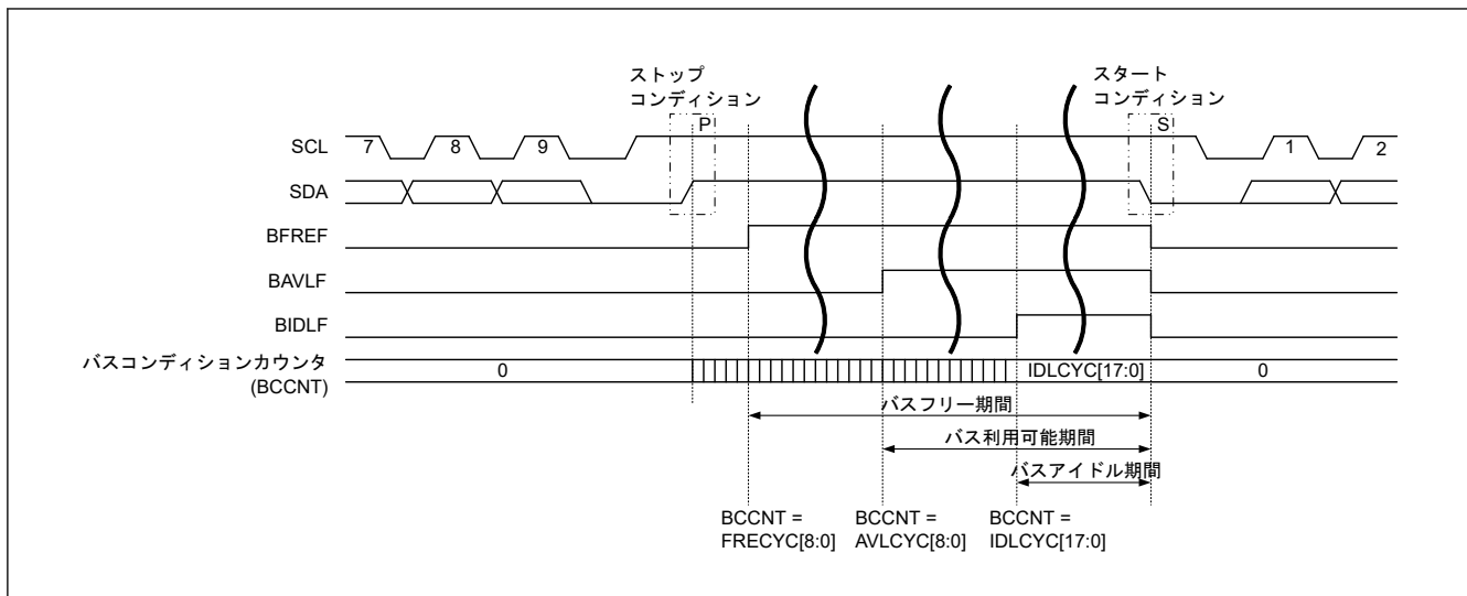
図 33.78 バス状態
