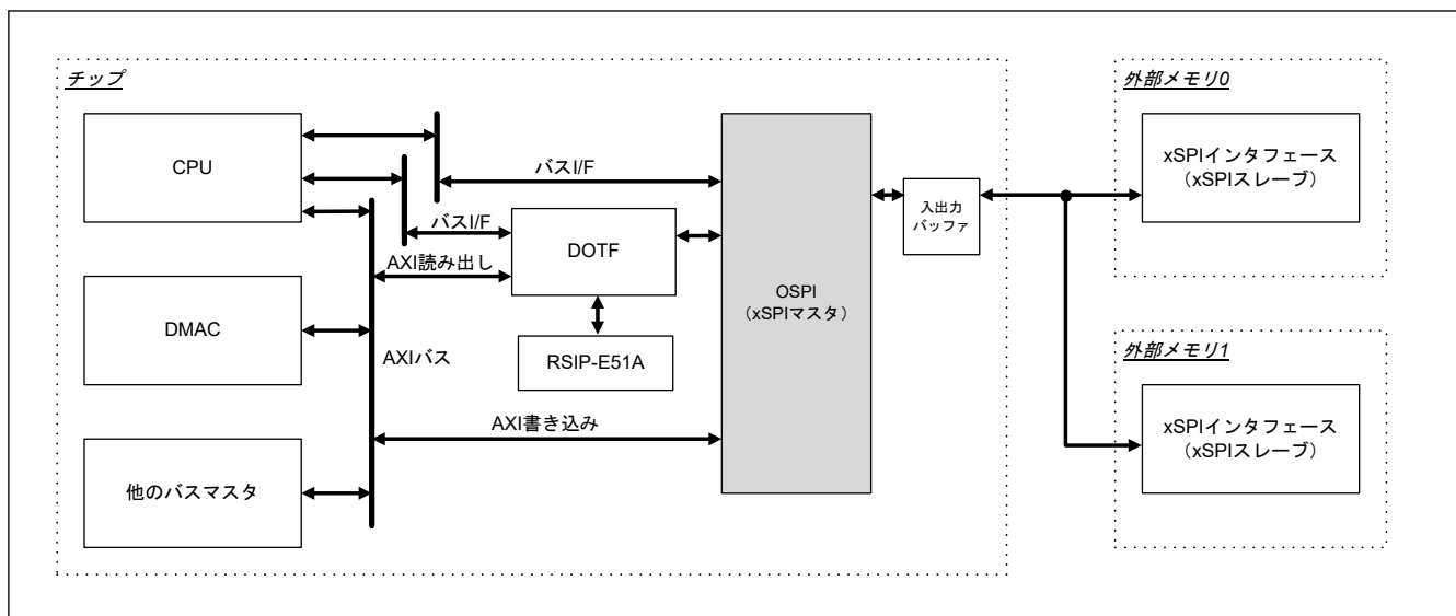
図 37.1 ブロック図
