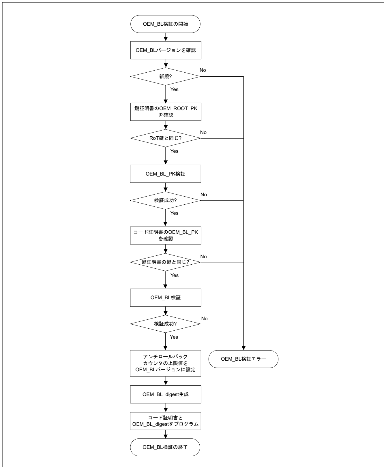
図 43.11 OEM_BL 検証フロー (シリアルプログラミングモード)
