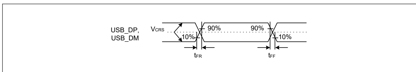
図 55.110 フルスピードモードにおける USB_DP、USB_DM の出カタイミング
