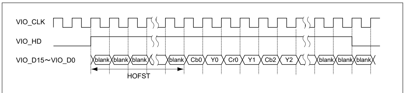
図 53.19 水平オフセット
