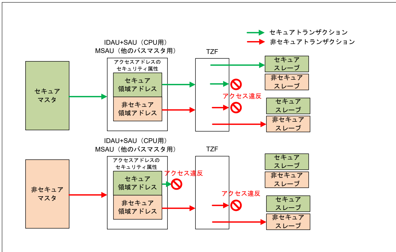
図 43.1 各マスタが発行できるトランザクション
