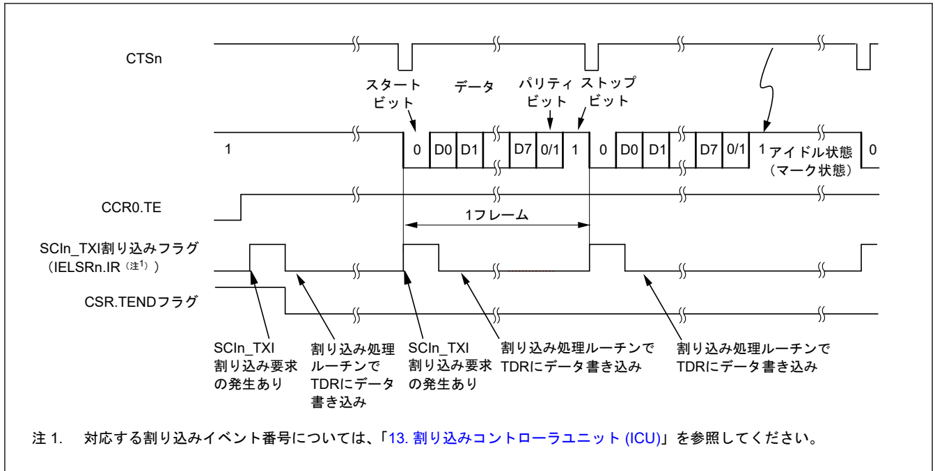
図 31.13 調歩同期式モードにおけるシリアル送信の動作例 (2) (8 ビットデータ/パリティあり/1ストップビット/CTS 機能使用/送信開始時)
