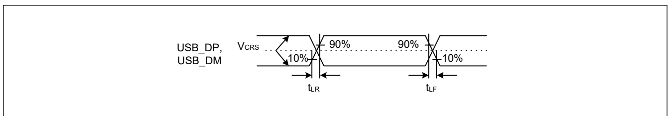
図 55.108 Low-speed モードにおける USB_DP、USB_DM の出カタイミング
