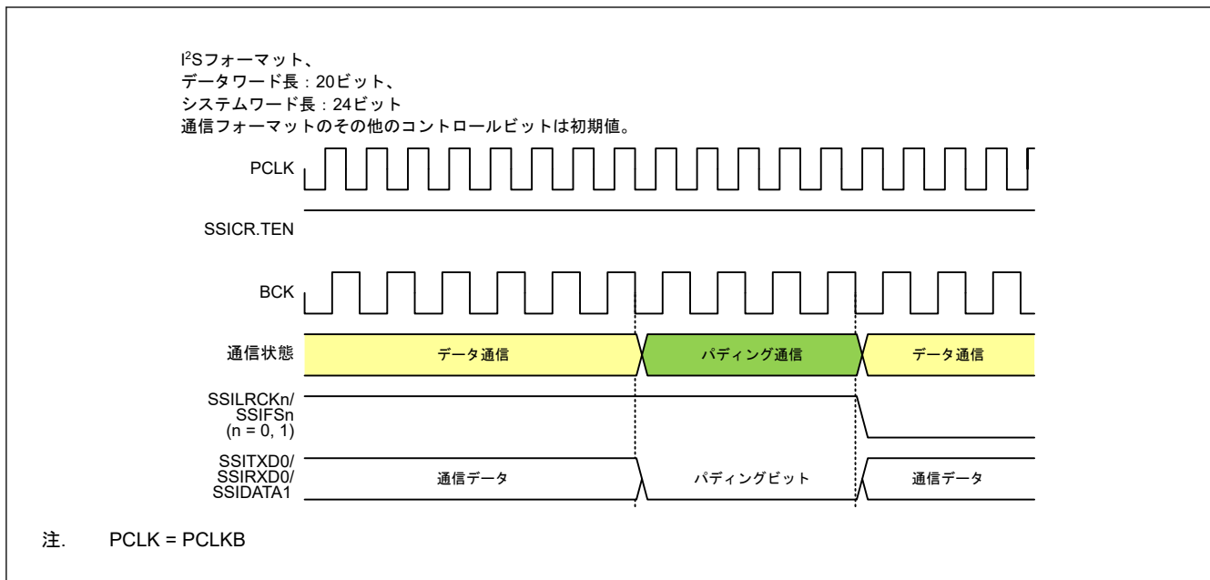
図 39.49 データ通信からパディング通信への遷移
