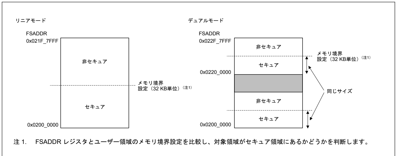
図 52.39 ユーザー領域内のセキュア領域と非セキュア領域 (セキュアエイリアスの場合)
