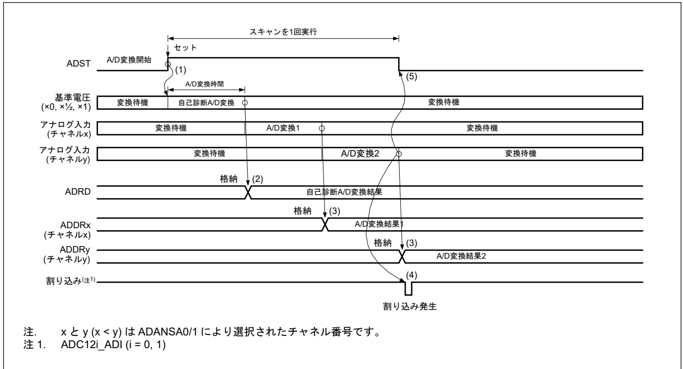
図 45.11 シングルスキャンモードの基本動作例（アナログ入力（チャンネル x、y）選択+自己診断）
