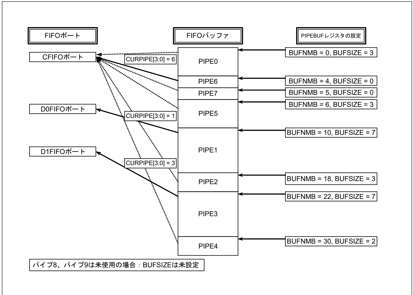
図 30.11 FIFO バッファのメモリマップ例
