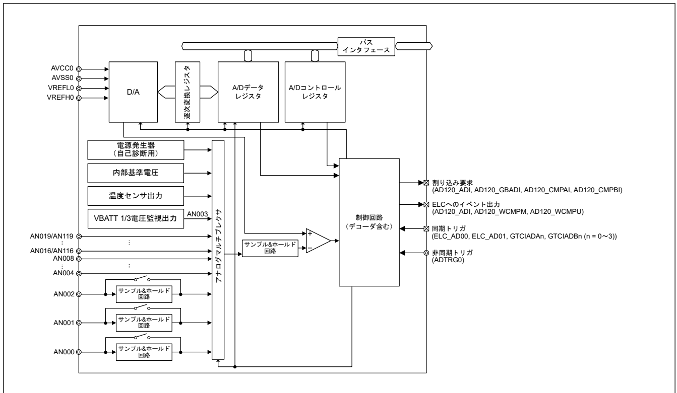
図 45.1 ADC12 のブロック図 (ユニット 0)
