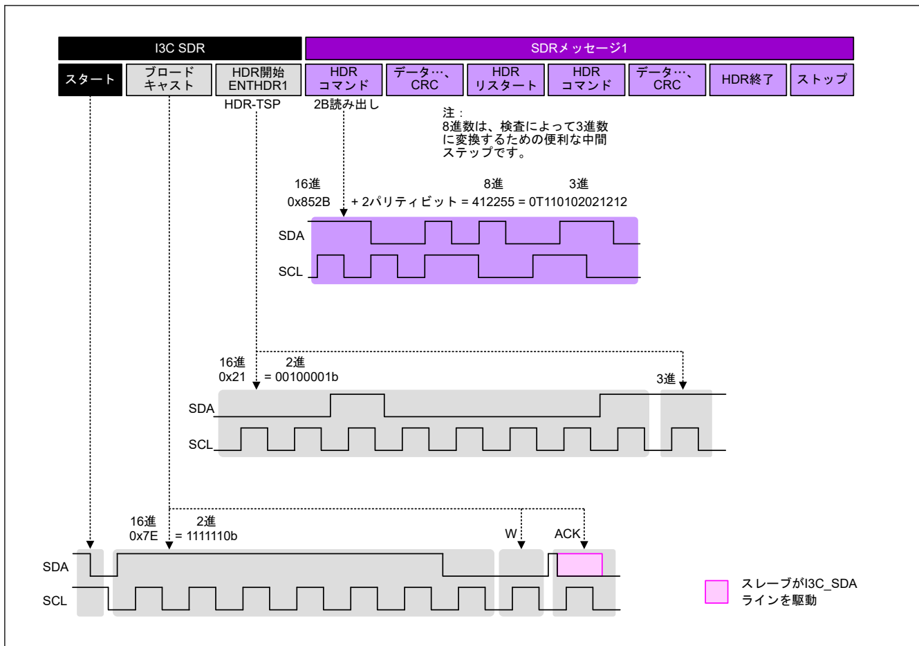
図 33.77 HDR-TSP プロトコルを使用した通信の例
