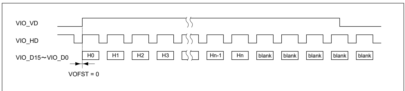
図 53.18 VD がデータイネーブル信号の場合のタイミング
