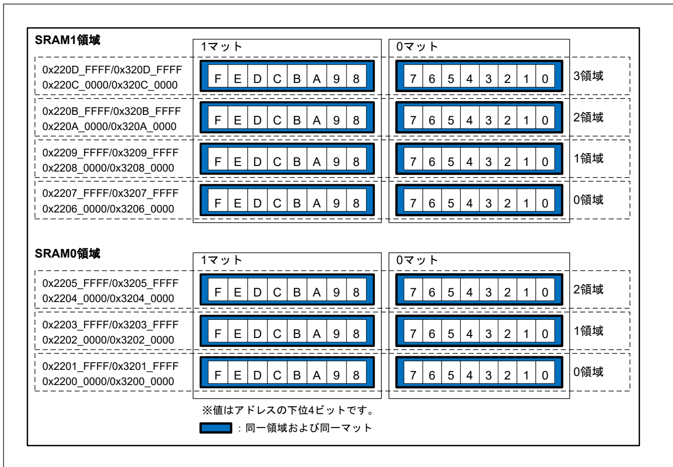
図 50.1 各 SRAM のマット設定
