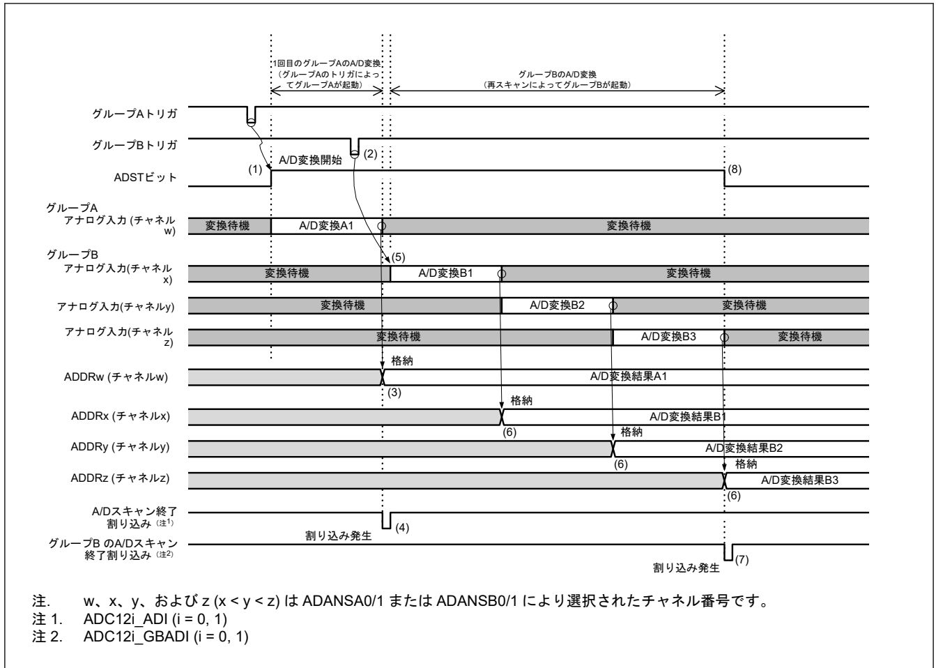
図 45.29 グループ優先動作の例 1-3 : グループ A スキャン中のグループ B トリガ入力、再スキャンあり (ADGSPCR.GBRSCN = 1、ADGSPCR.GBRP = 0、および ADGSPCR.LGRRS = 0 の場合)
