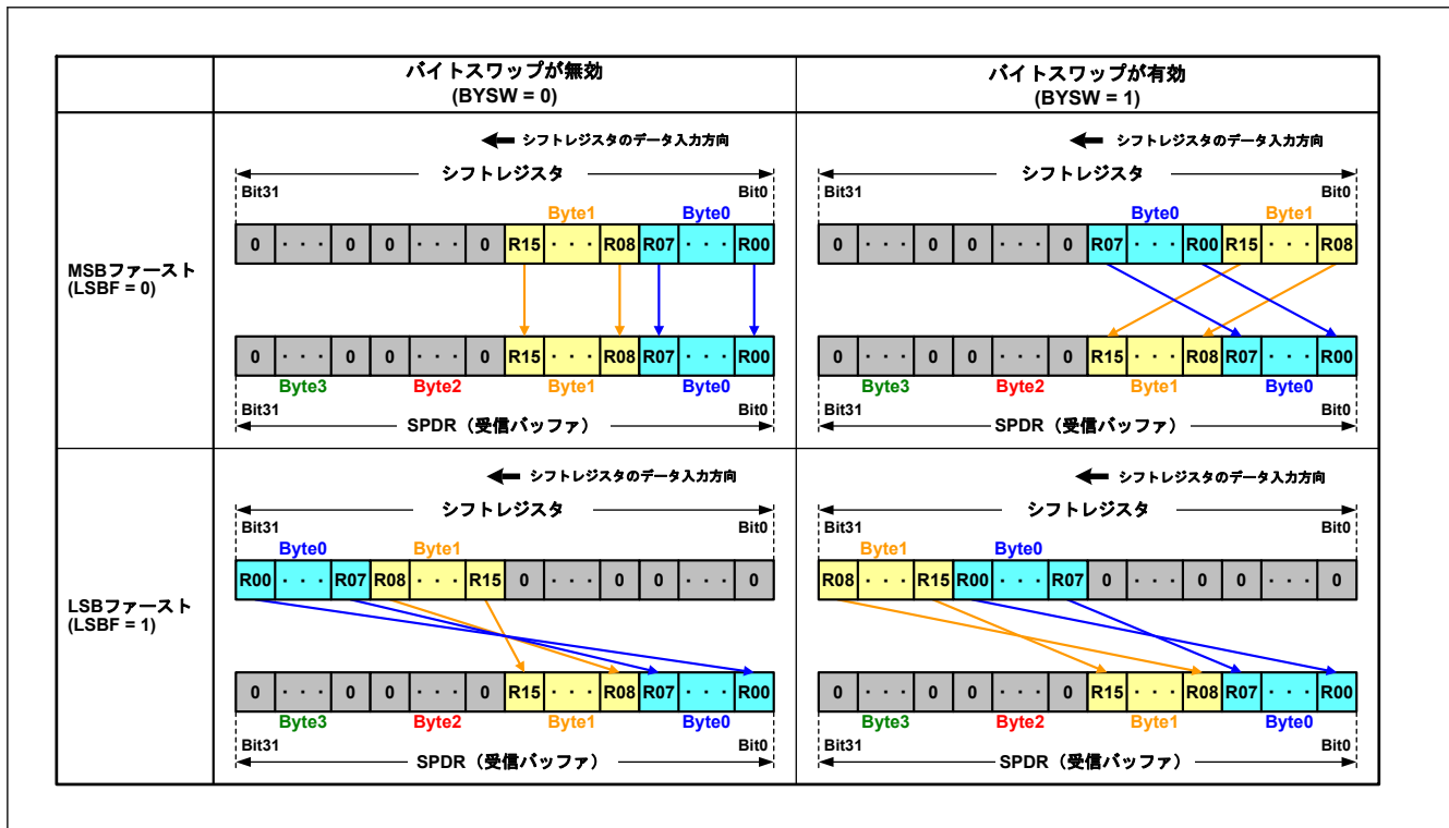
図 36.26 MSB/LSB 転送でのバイトスワップ (16 ビット)
