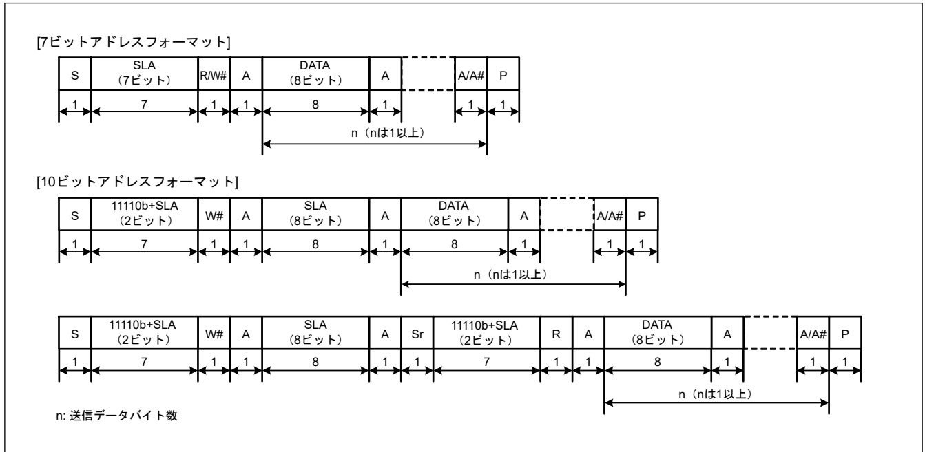
図 33.69 I 2 C バスフォーマット
