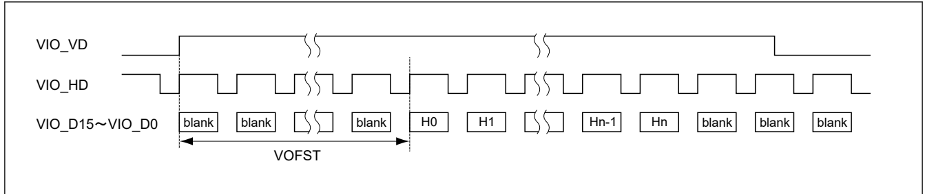
図 53.17 垂直オフセット
