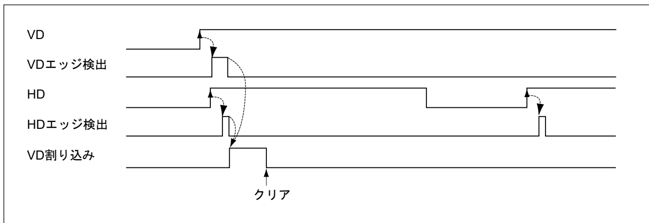
図 53.15 VD と HD が正極性の場合の VIO_VD および VIO_HD 信号と VD 割り込みの関係 (画像キャプチャモードおよびデータ同期取り込みモードの場合)
