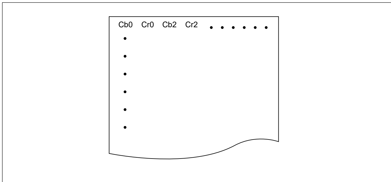
図 53.52 色差成分のメモリ格納イメージ
