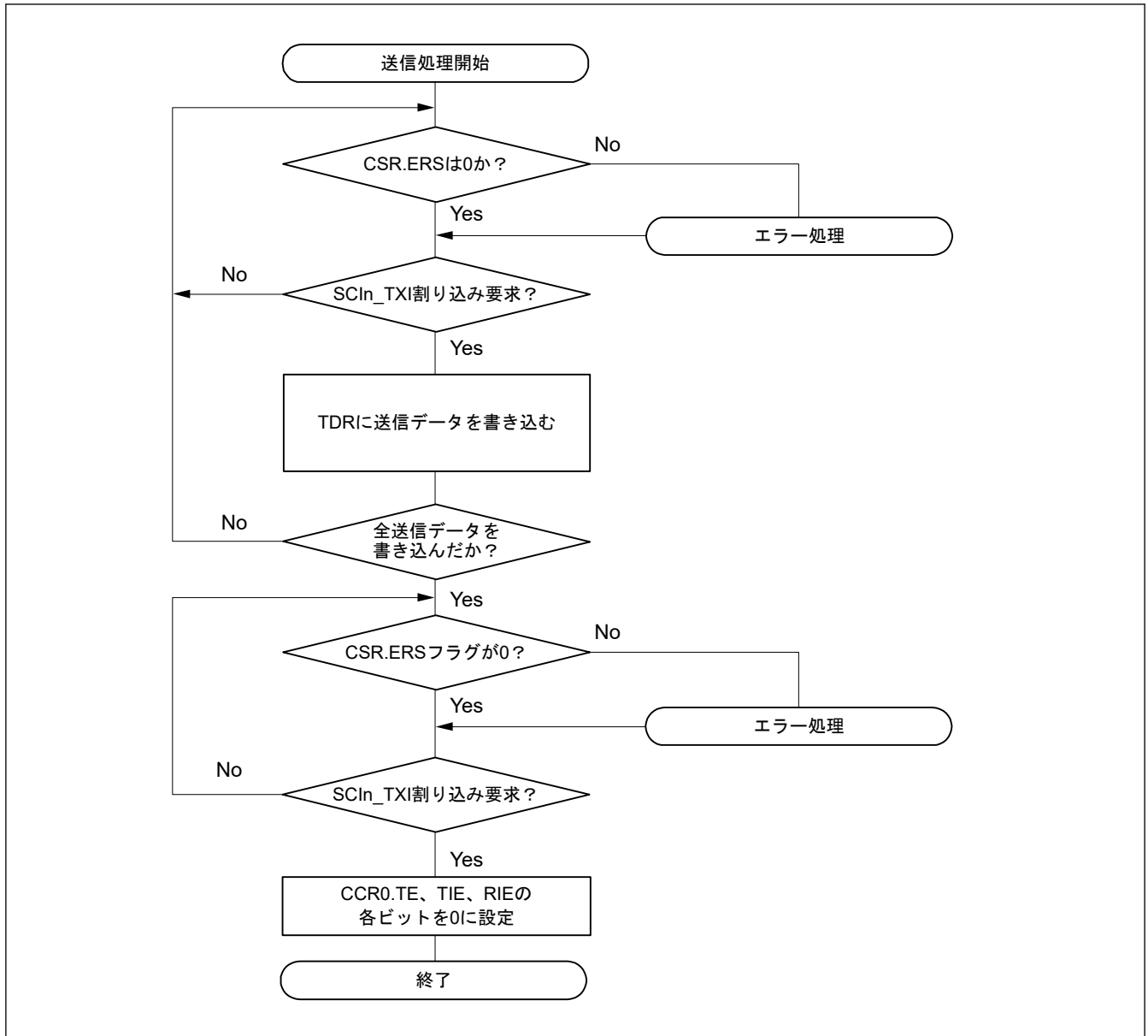
図 31.82 スマートカードインタフェース送信のフローチャート例
