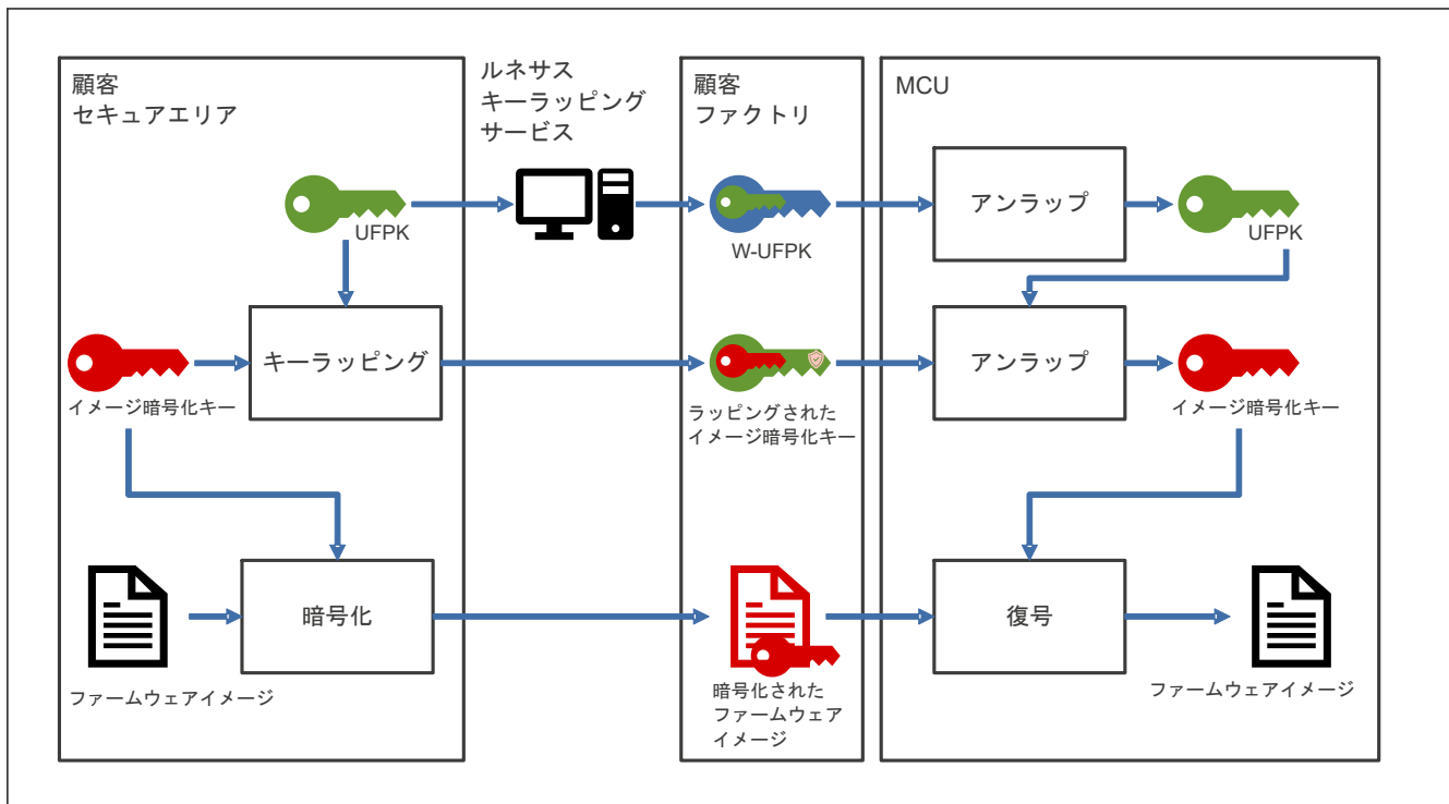
図 43.10 セキュアファクトリ暗号化イメージプログラミング
