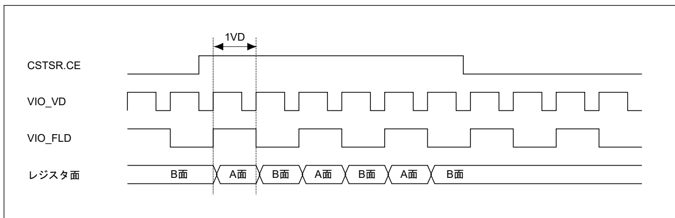
図 53.31 RVS = 1 のときのレジスタ面切り替えタイミング
