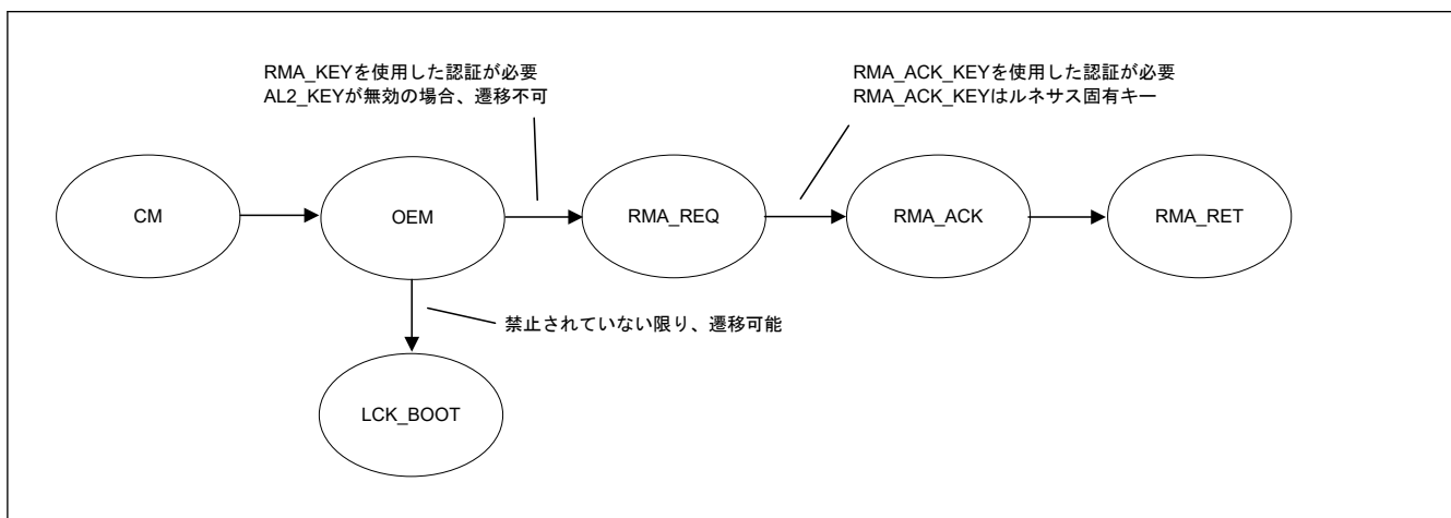
図 43.7 デバイスライフサイクル状態
