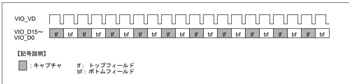
図 53.27 インターレース入力方式での片フィールド連続キャプチャ（起動直後の画像がトップフィールドの場合 (FCI[1:0] = 00b)
