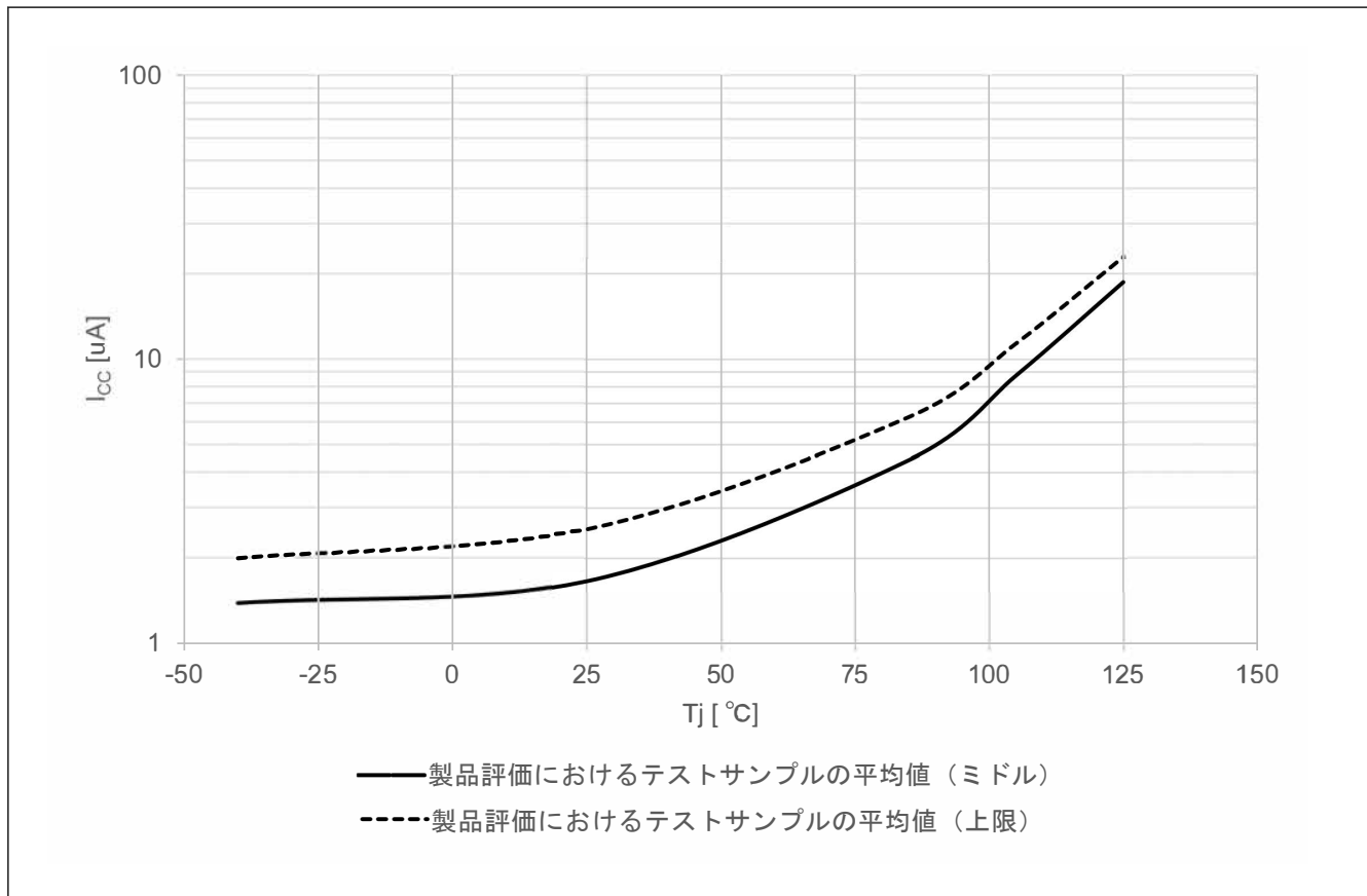
図 55.6 ディープソフトウェアスタンバイモード2における温度依存性 (参考データ)
