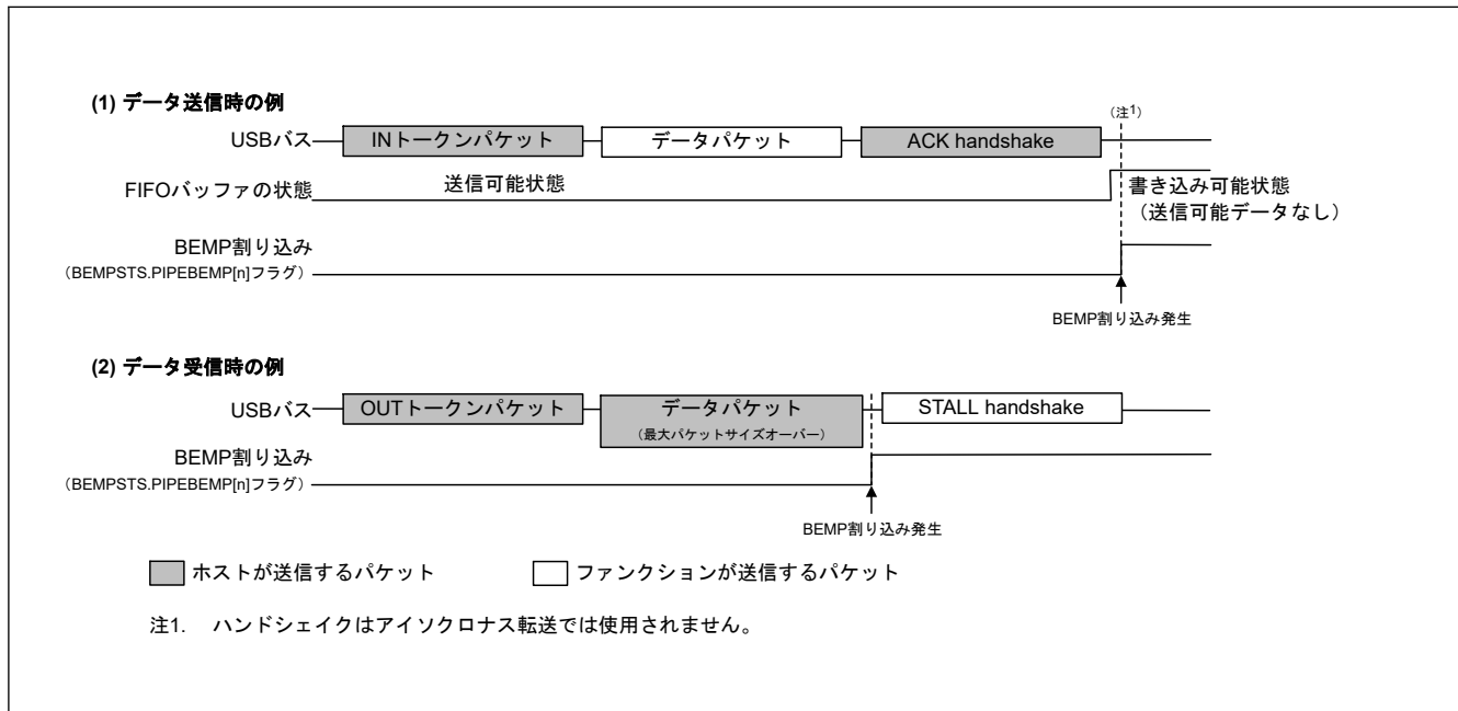
図 30.7 デバイスコントローラモード時の BEMP 割り込みの発生タイミング
