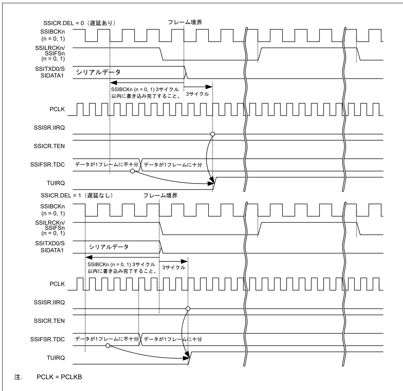
図 39.20 TUIRQ 設定タイミング (通信継続時)
