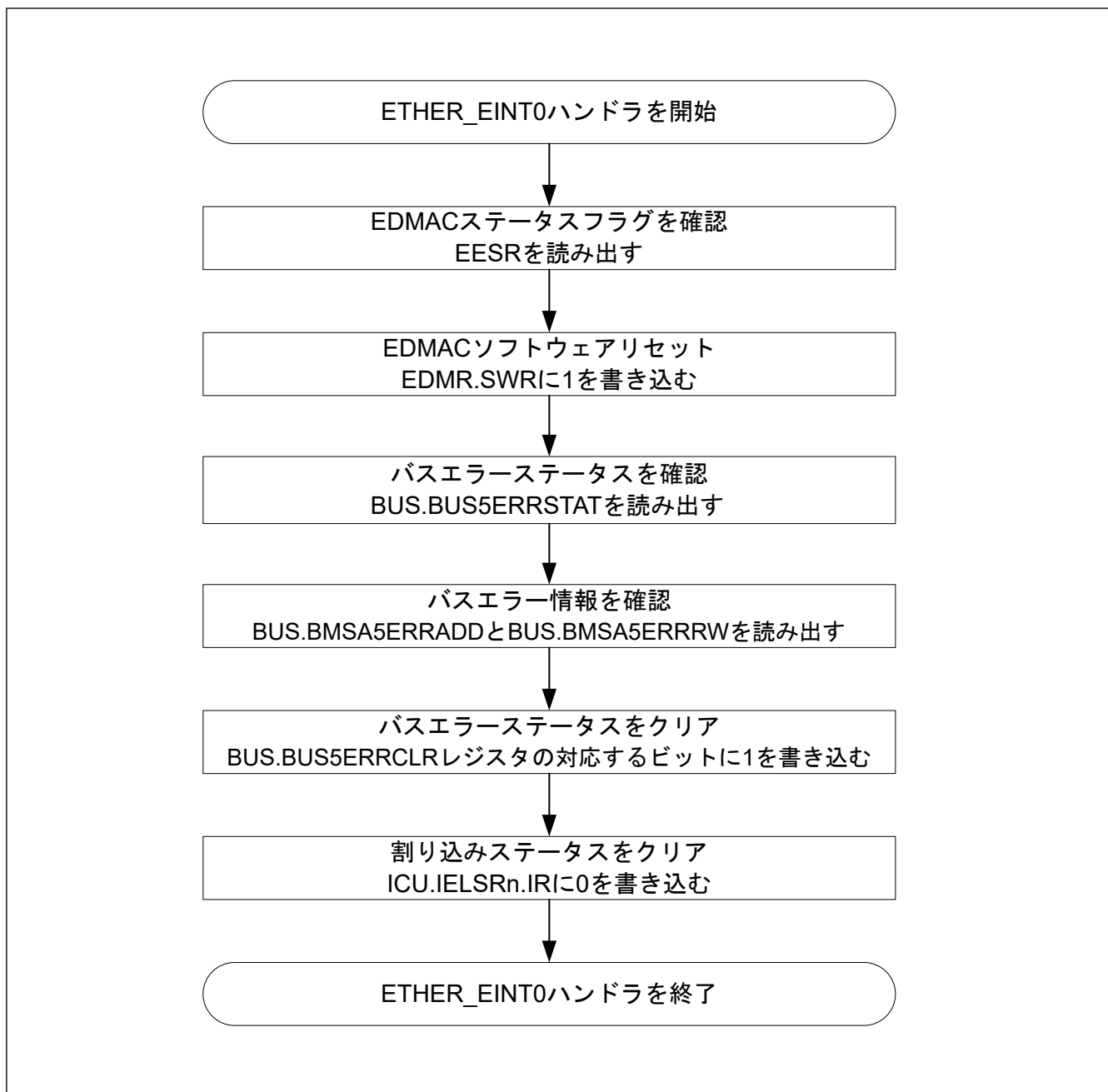
図 28.10 ETHER_EINT0 ハンドラにおけるバス転送エラーの処理
