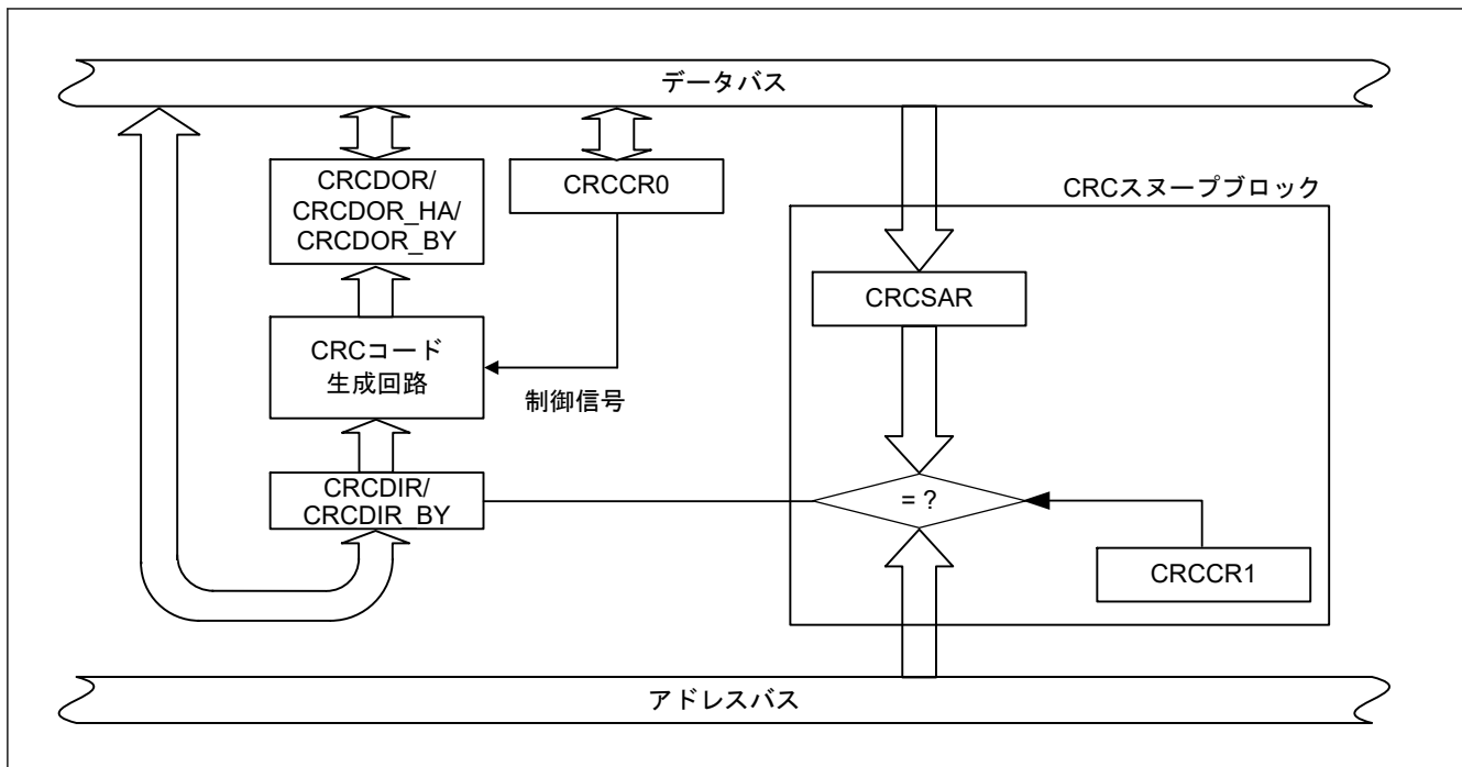
図 41.1 CRC 演算器のブロック図
