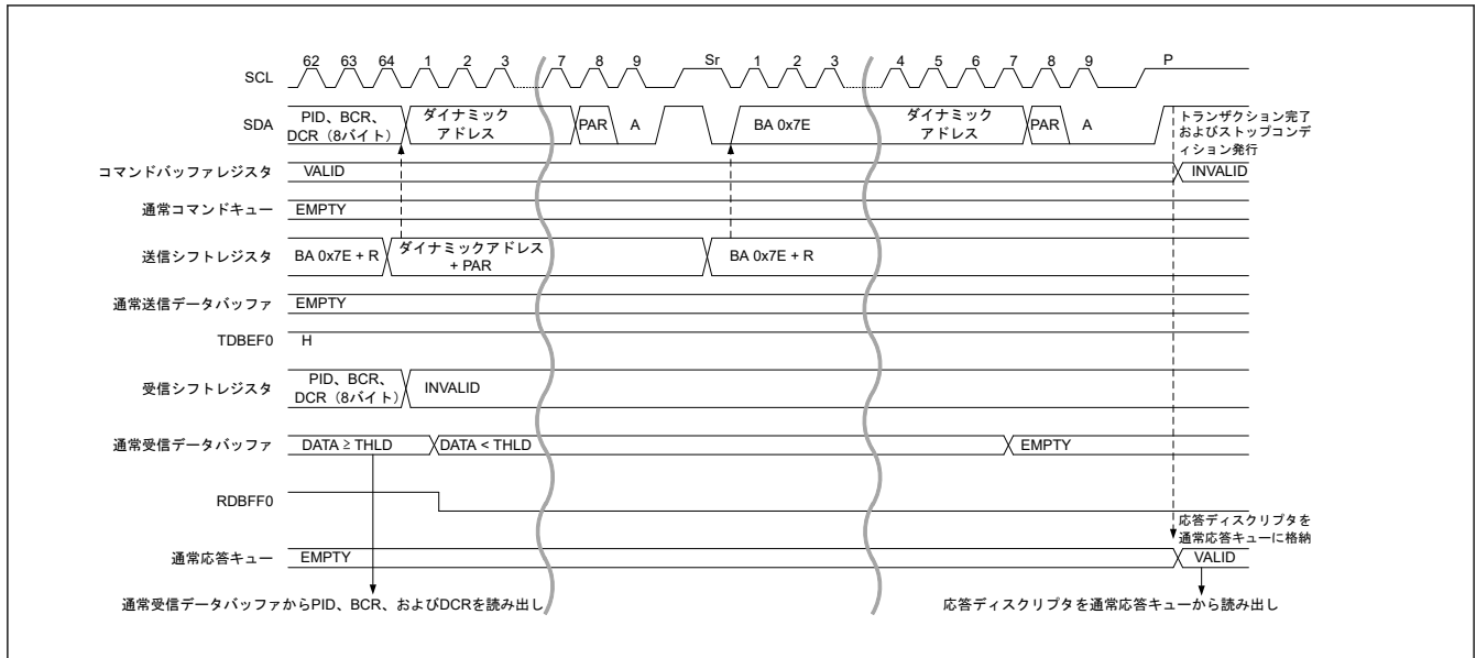
図 33.14 ダイナミックアドレス配置手順 (ENTDAA CCC) タイミング (3/3)
