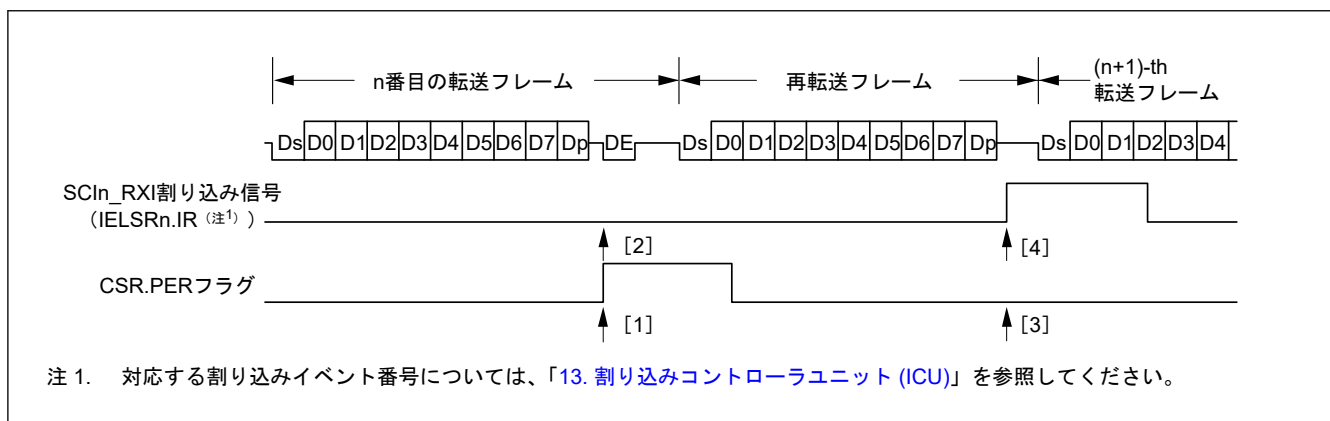
図 31.83 スマートカードインタフェース受信モードでの再転送動作
