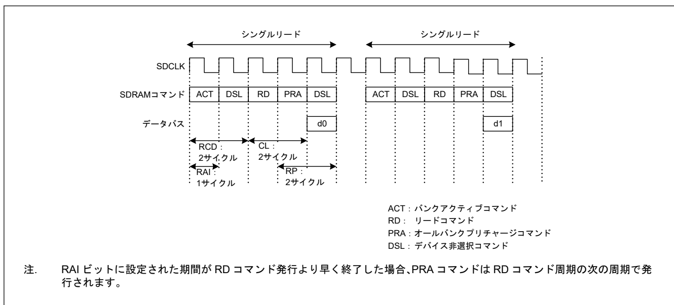
図 14.53 シングルリードタイミング例 (2)
