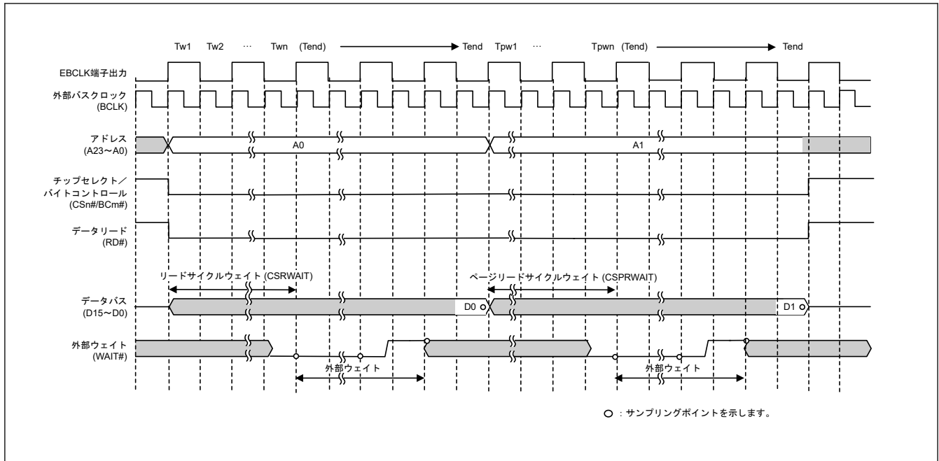
図 14.25 外部ウェイトタイミング例 (16 ビットバス空間に対するページリードアクセス、EBCLK 端子出力選択ビットで BCLK の 2 分周を選択した場合) (n = 0~7, m = 0, 1)
