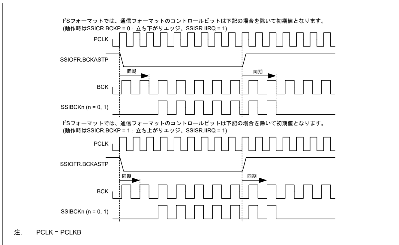
図 39.45 SSIOFR.BCKASTP による SSIBCKn (n = 0, 1) 停止の例
