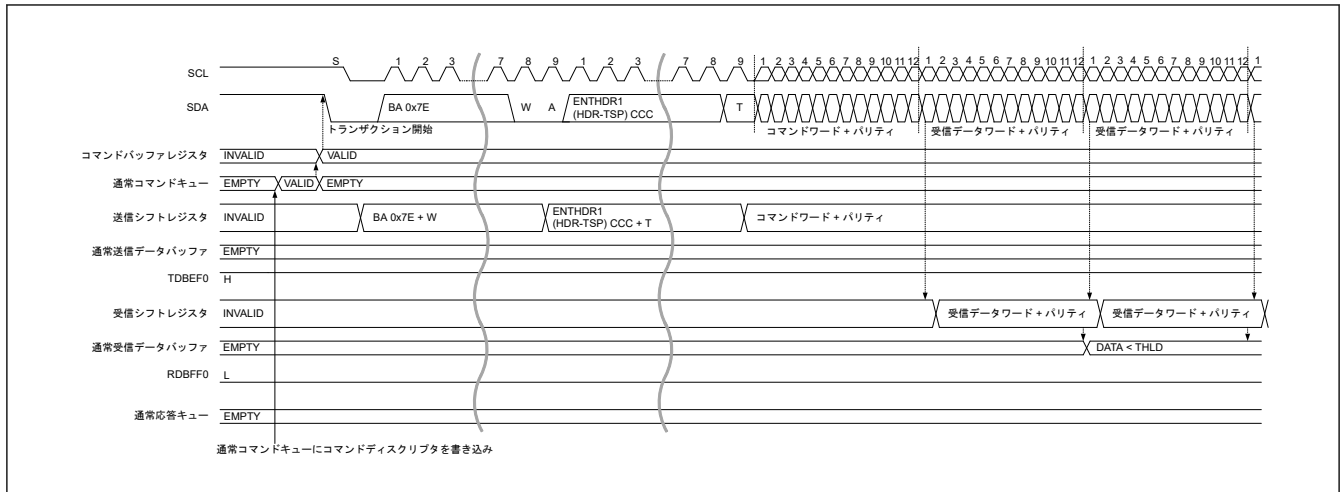
図 33.32 HDR データ読み出し転送 (HDR-TSP、TSL) タイミング (1/2)
