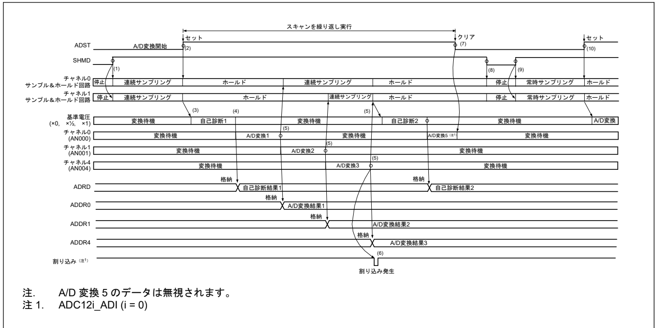
図 45.22 連続スキャンモードの動作例 (チャンネル専用サンプル&ホールド回路使用、AN000、AN001、および AN004 選択+自己診断、連続サンプリング有効)
