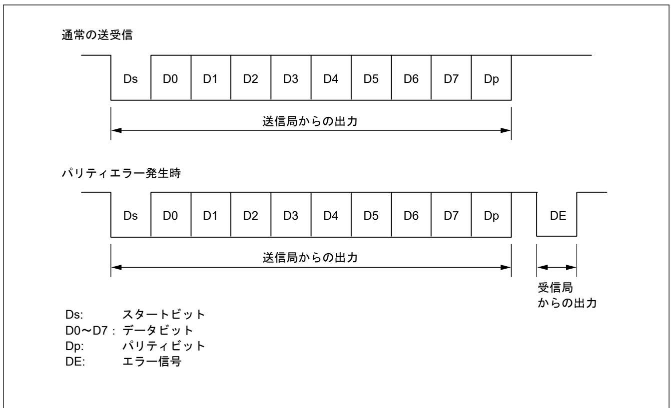
図 31.75 スマートカードインタフェースモードにおけるデータフォーマット
