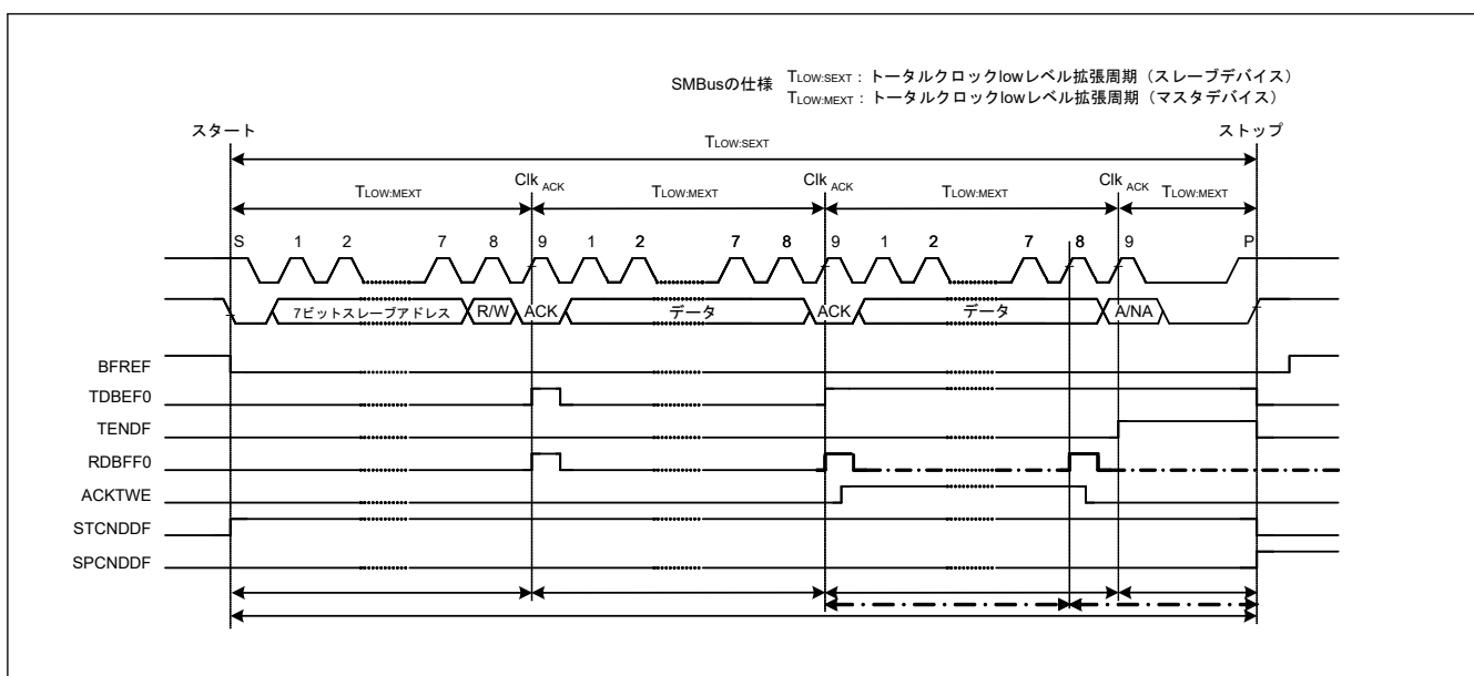
図 33.114 SMBus タイムアウト測定
