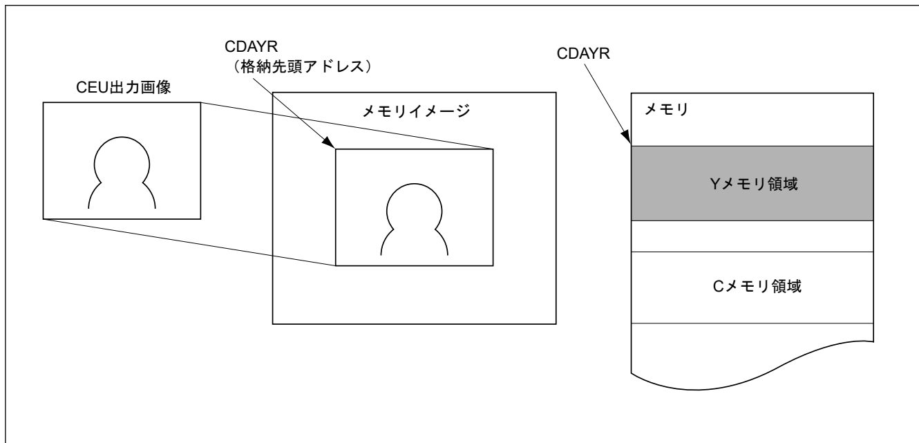
図 53.34 キャプチャ画像と輝度成分メモリ領域の関係
