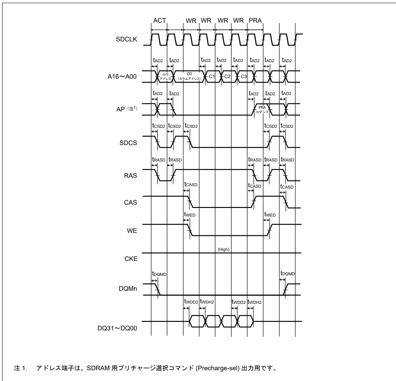
図 55.38 SDRAM マルチライトのタイミング
