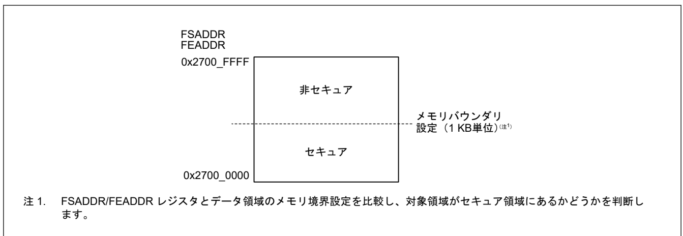
図 52.40 データ領域内のセキュア領域と非セキュア領域 (セキュアエイリアスの場合)
