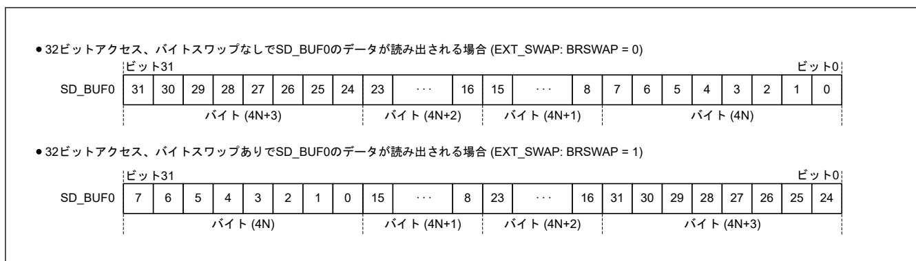
図 40.6 SD_BUF0 からの読み出し
