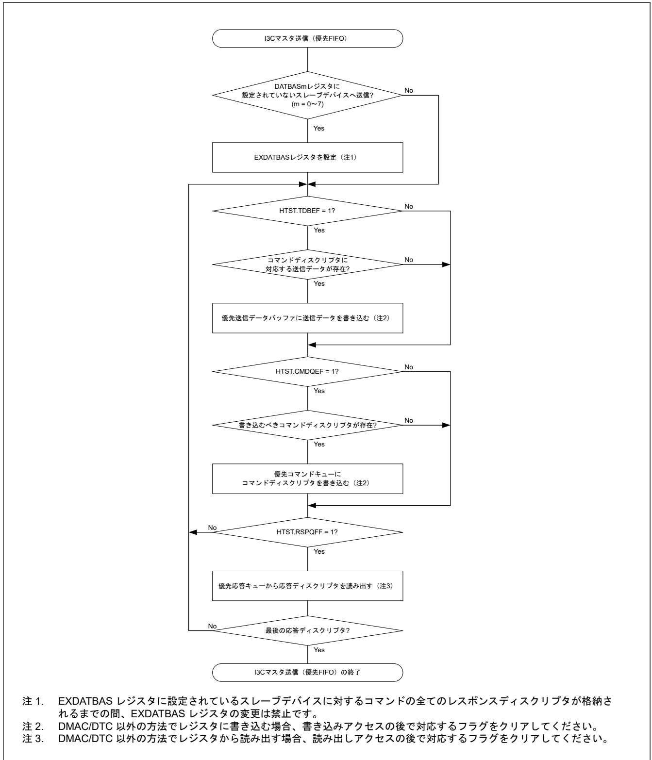
図 33.148 I3C マスタ送信のフローチャート例（優先 FIFO バッファ転送）
