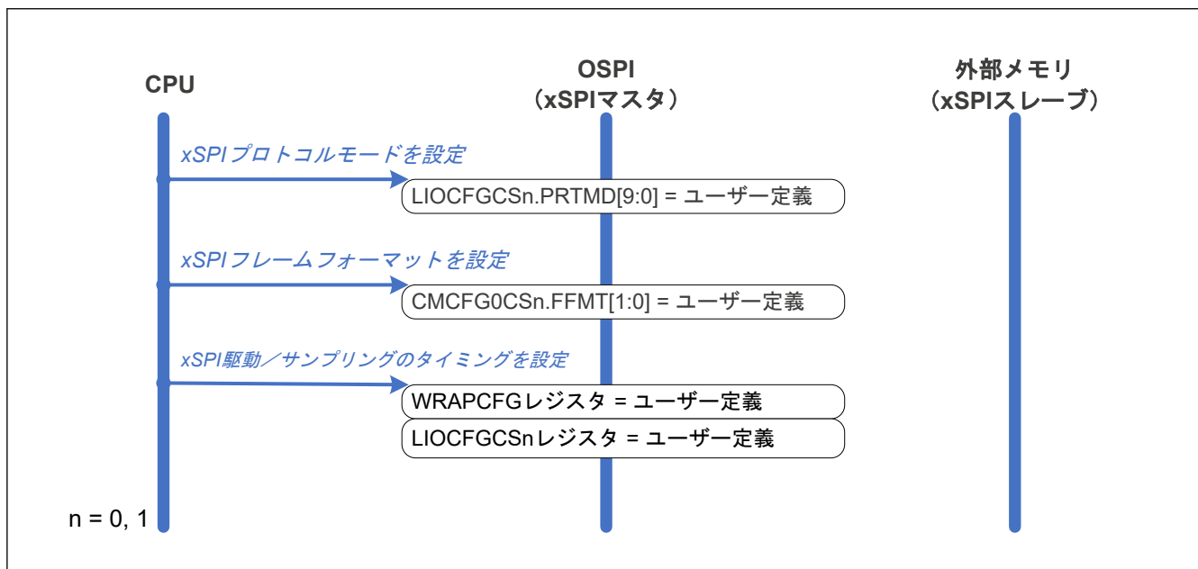
図 37.22 設定のフロー
