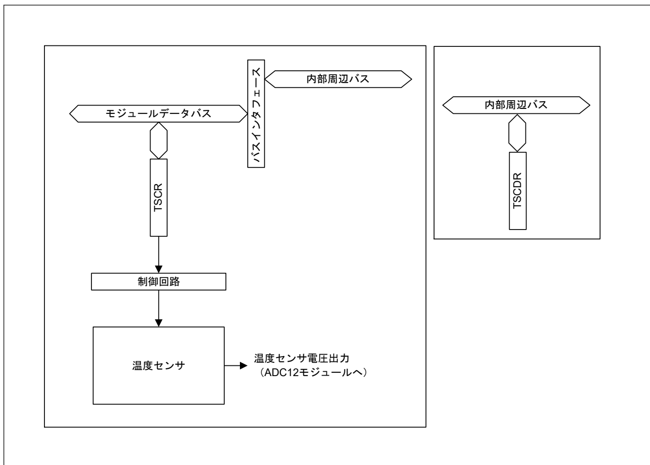
図 47.1 TSN のブロック図
