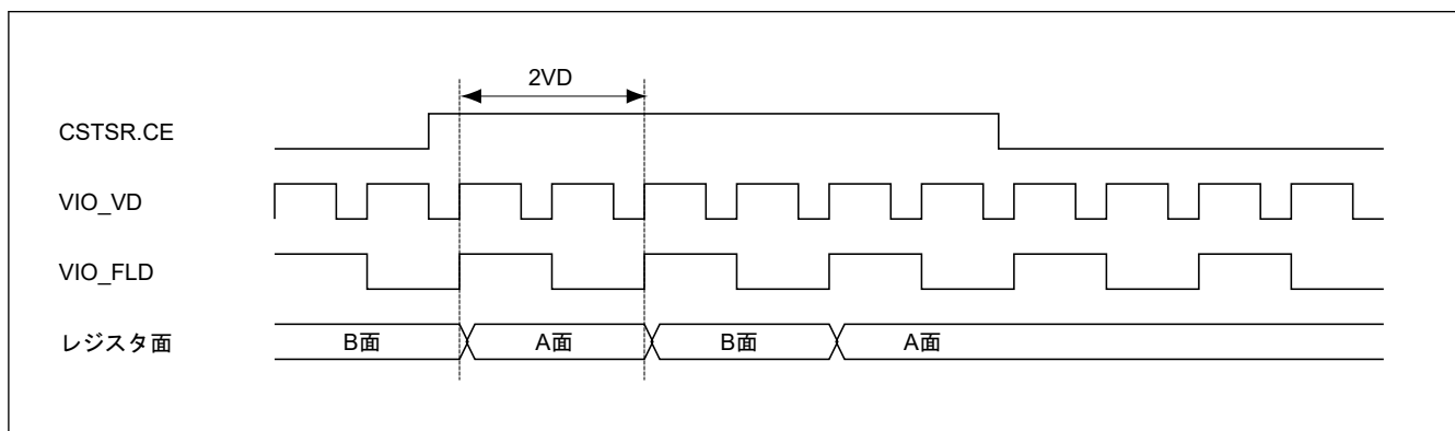
図 53.30 RVS = 0 のときのレジスタ面切り替えタイミング
