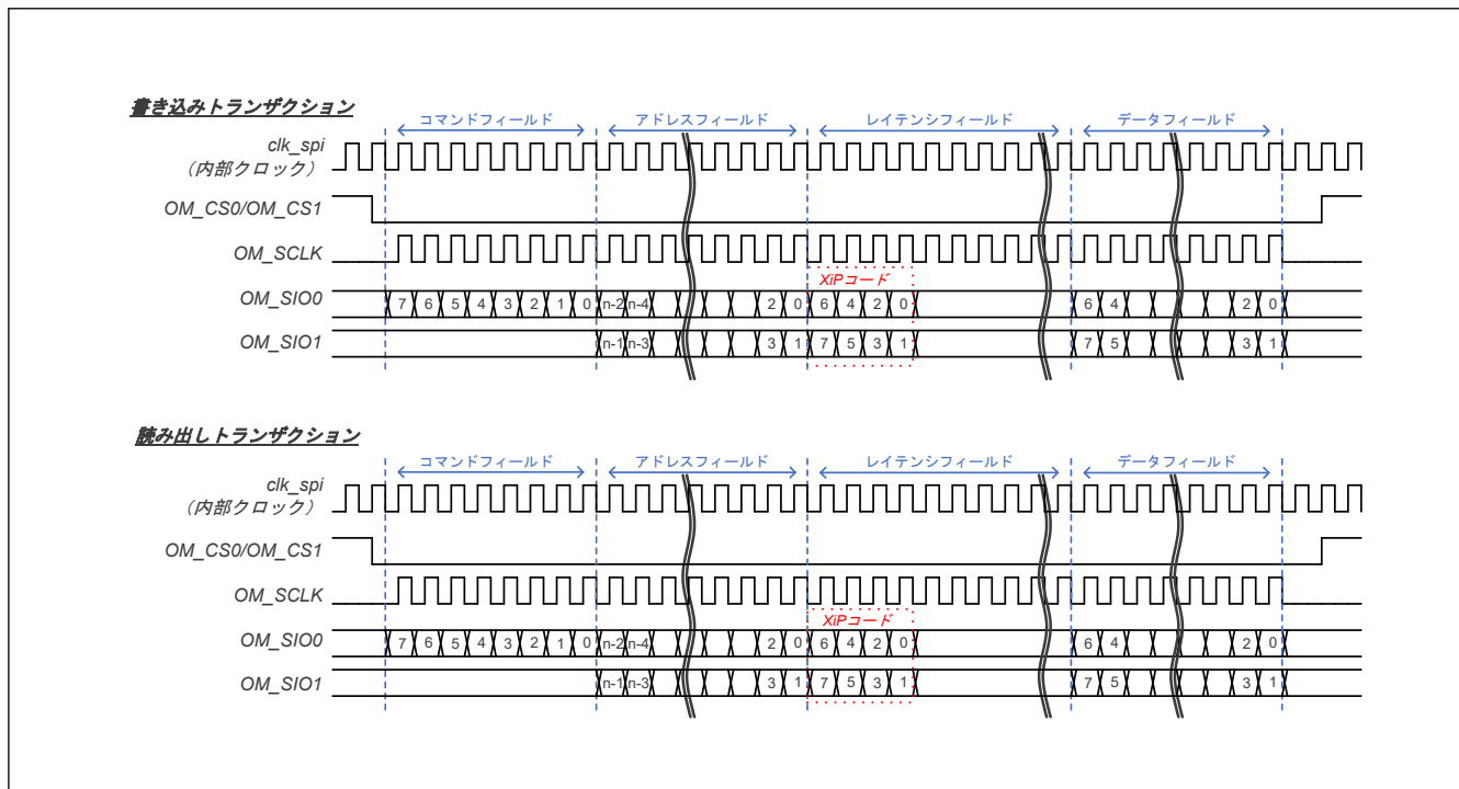
図 37.4 1S-2S-2S のタイミングチャート
