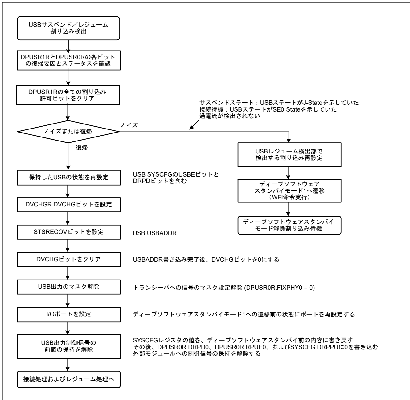
図 29.8 ホストコントローラ機能選択時におけるディープソフトウェアスタンバイモード1解除時のUSBFS設定フロー
