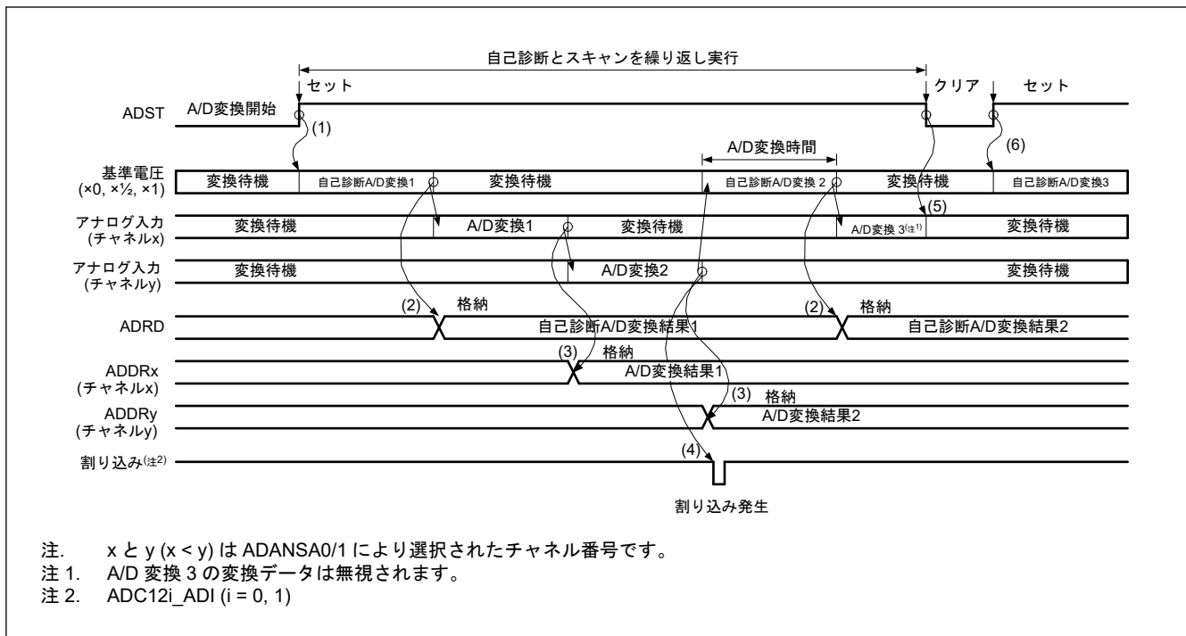
図 45.20 連続スキャンモードの基本動作例 (アナログ入力 (チャンネル x、y) 選択+自己診断)
