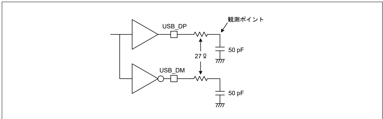
図 55.107 フルスピードモードにおける測定回路
