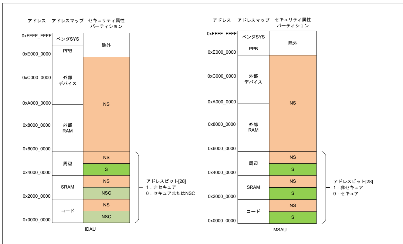
図 43.2 IDAU および MSAU の定義されたセキュリティマップ
