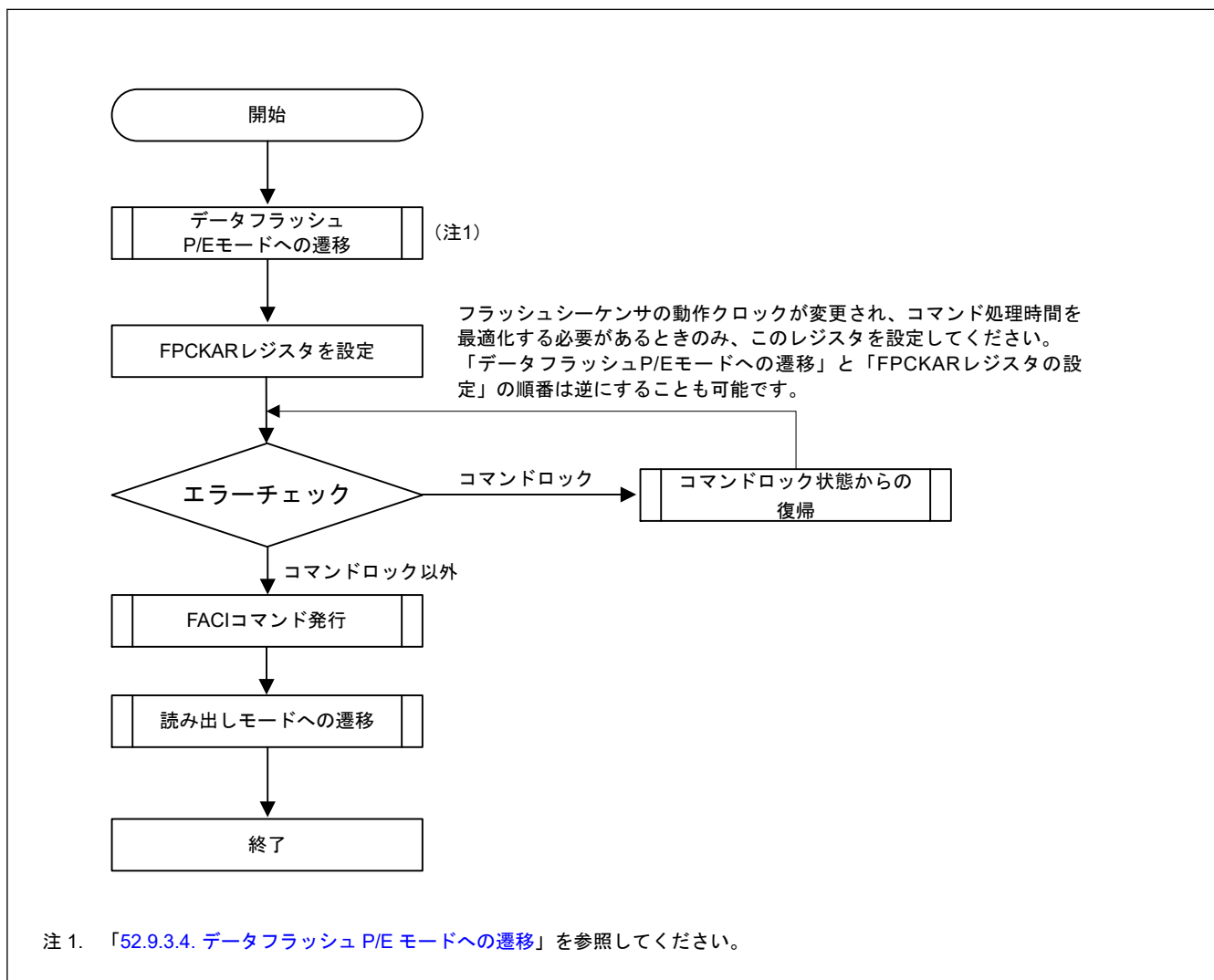
図 52.9 データフラッシュ P/E モードでのコマンド使用概要
