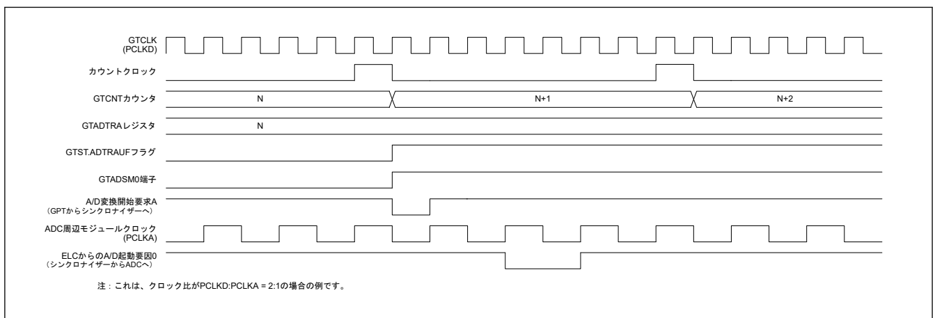
図 21.71 A/D 変換開始要求タイミング動作例
