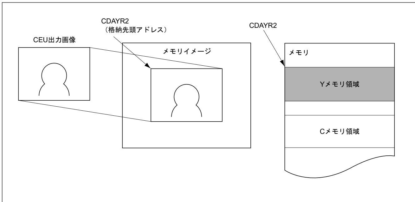
図 53.50 キャプチャ画像と輝度成分メモリ領域の関係
