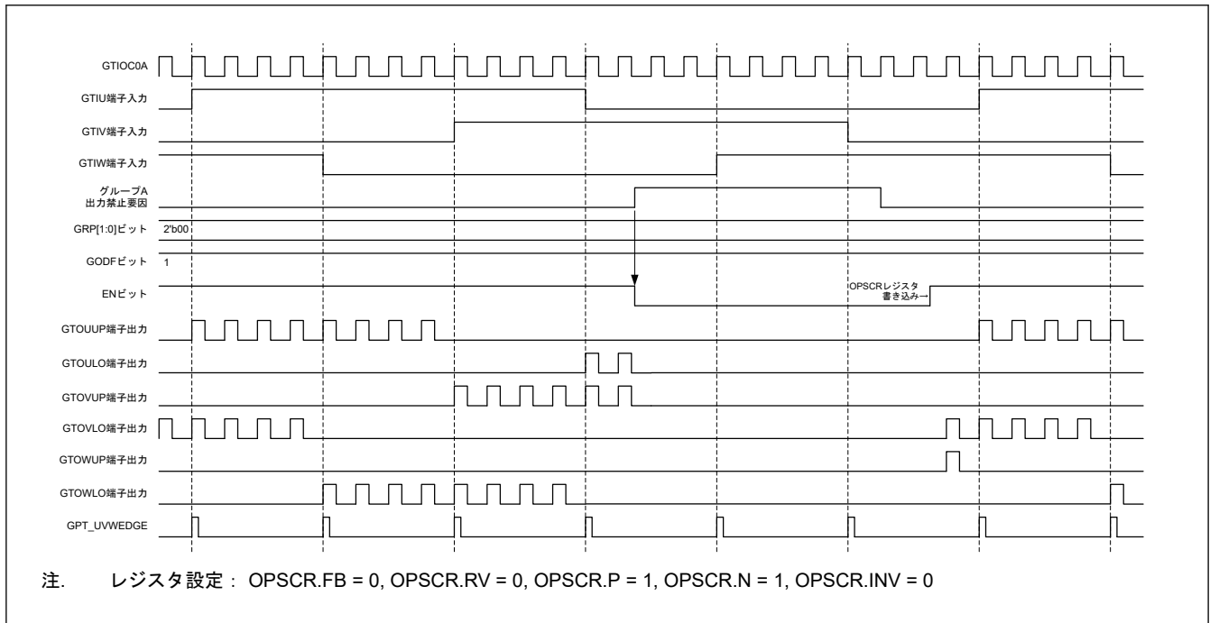
図 21.67 グループ出力禁止制御動作例
