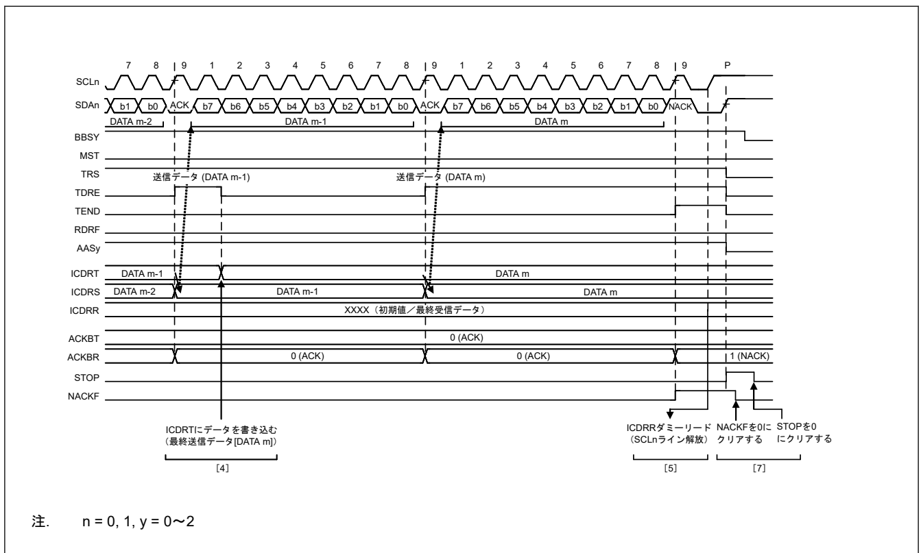
図 32.17 スレーブ送信の動作タイミング (2)
