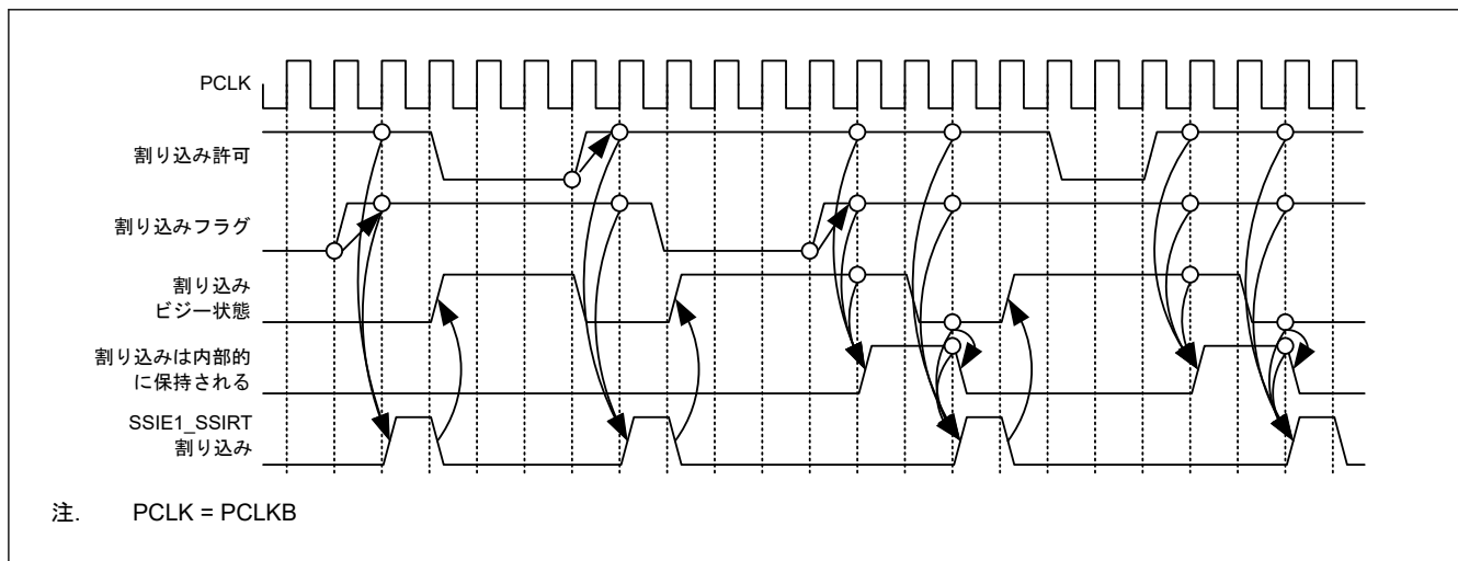
図 39.61 SSIE1_SSIRT 割り込みタイミング図
