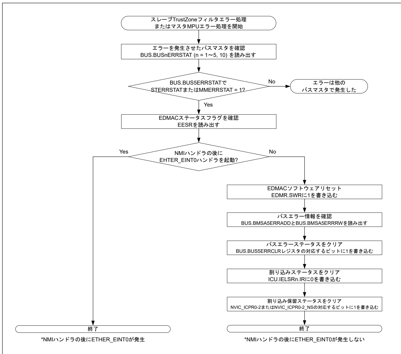
図 28.9 NMI ハンドラにおけるバス転送エラーの処理
