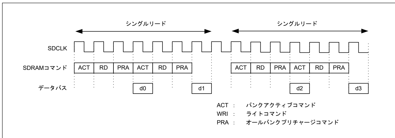
図 14.44 シングルリードのタイミング例 (SDAMOD.BE = 0 かつ SDTR.CL[2:0] = 010b : 2 サイクルでのバスマスタからのバースト転送)
