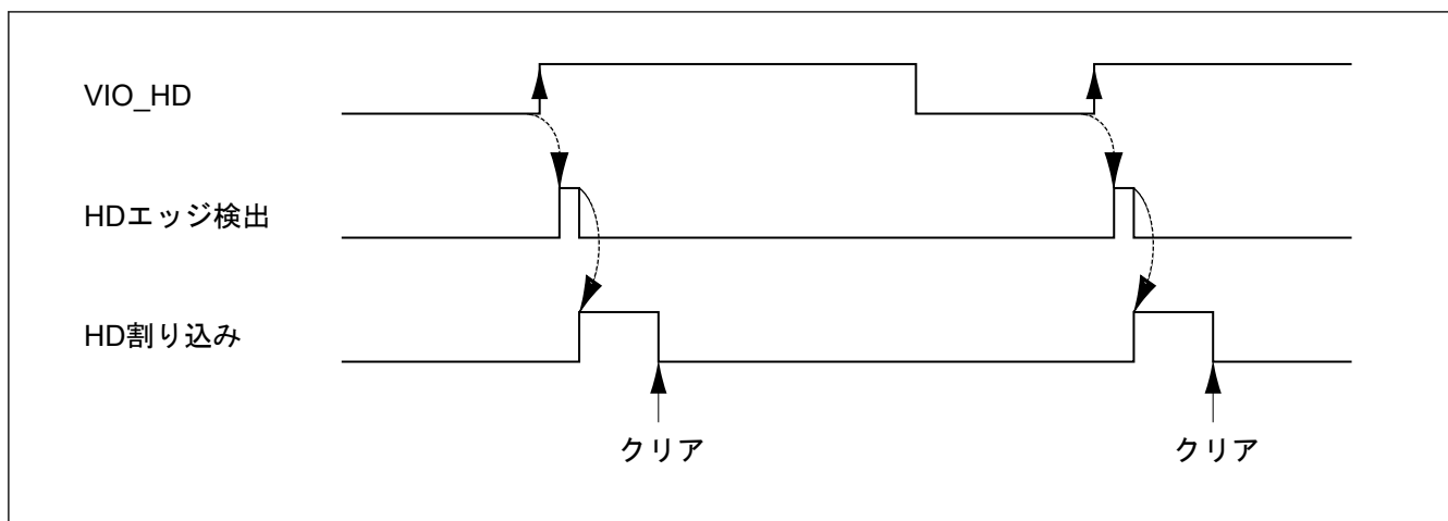
図 53.16 HD が正極性の場合の VIO_HD と HD 割り込みの関係
