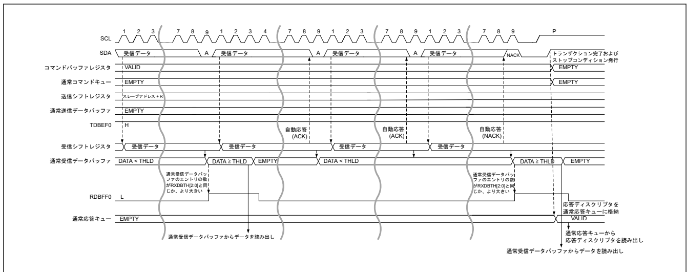
図 33.23 レガシー I 2 C メッセージデータ読み出し転送タイミング (2/2)
