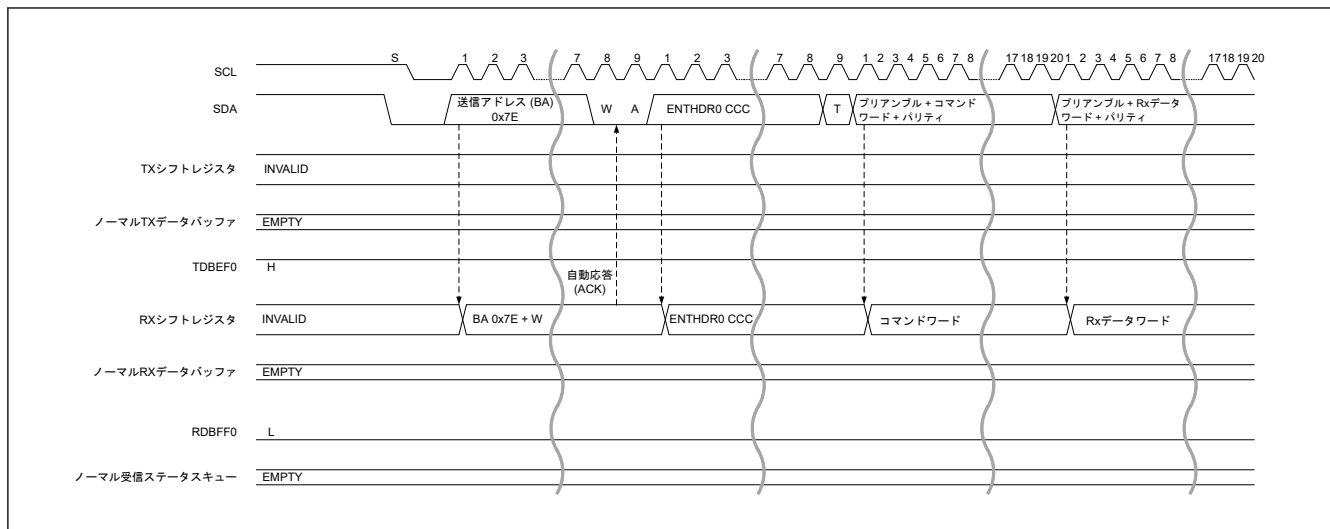
図 33.53 HDR データ書き込み転送 (HDR-DDR) タイミング (1/3)
