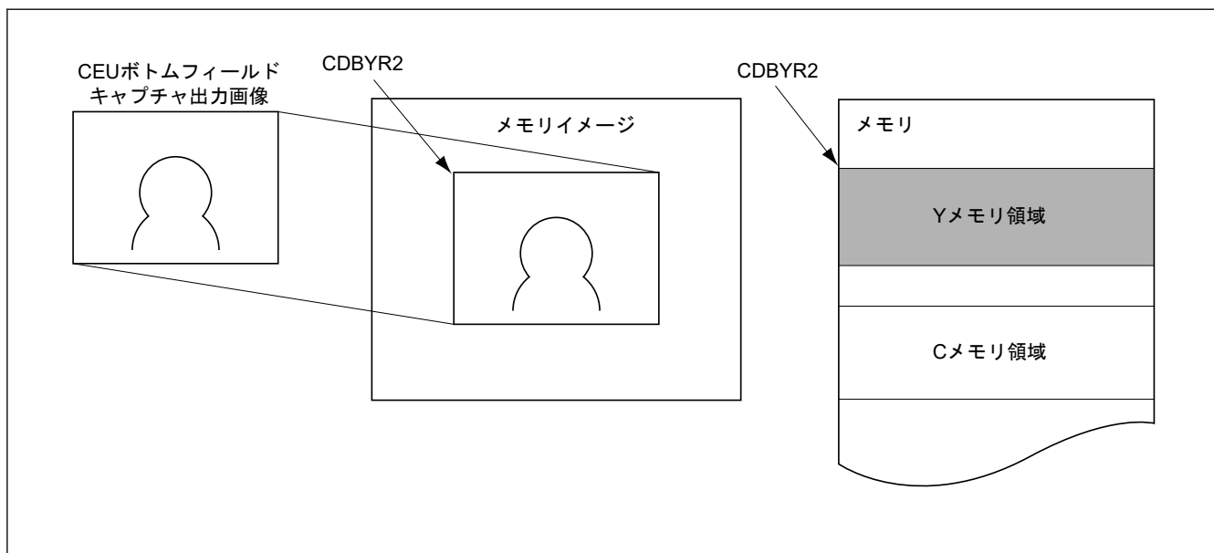
図 53.53 ボトムフィールドキャプチャ画像と輝度成分メモリ領域の関係
