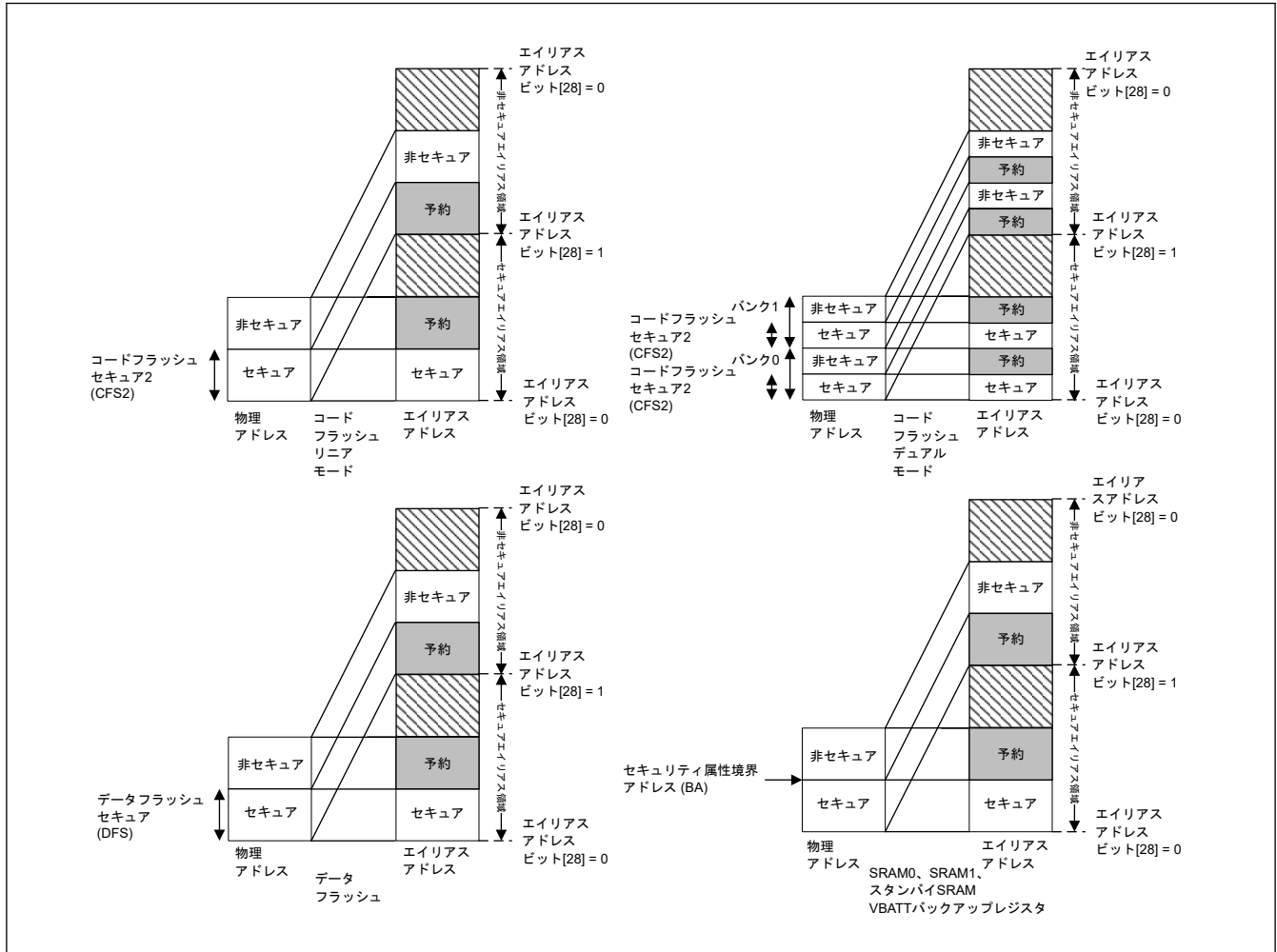
図 43.6 メモリマッピング
