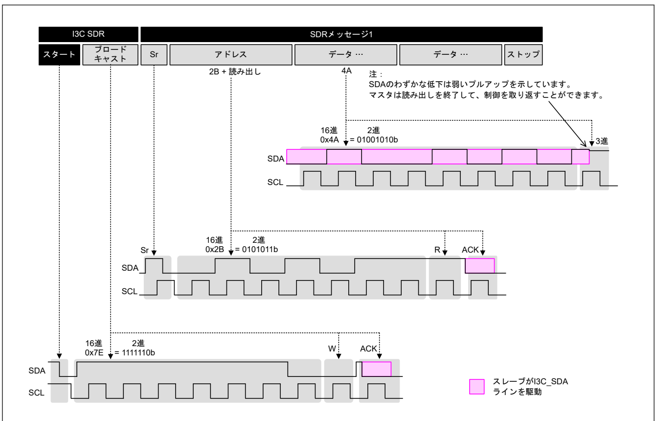
図 33.71 ブロードキャスト (0x7E) を含む I3C SDR コーディングを使用した通信の例
