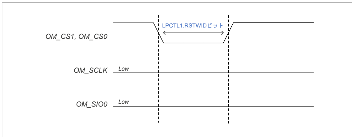
図 37.21 CS のみパターン
