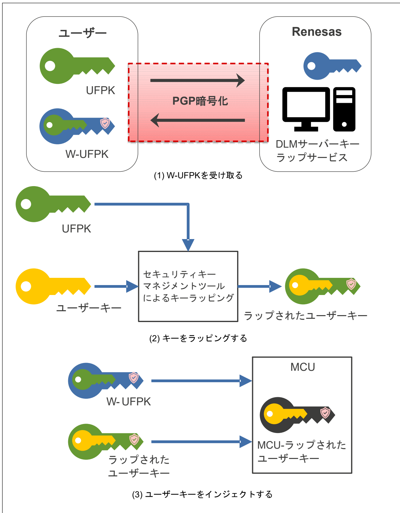
図 43.9 キーインジェクション
