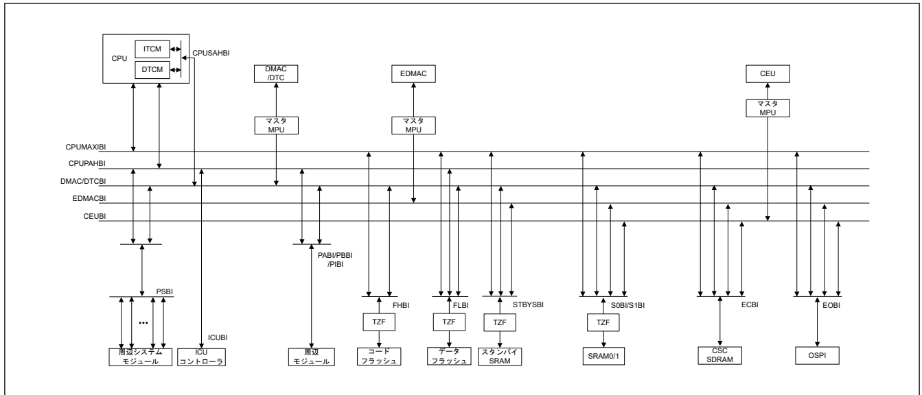
図 14.1 システムバスの接続
