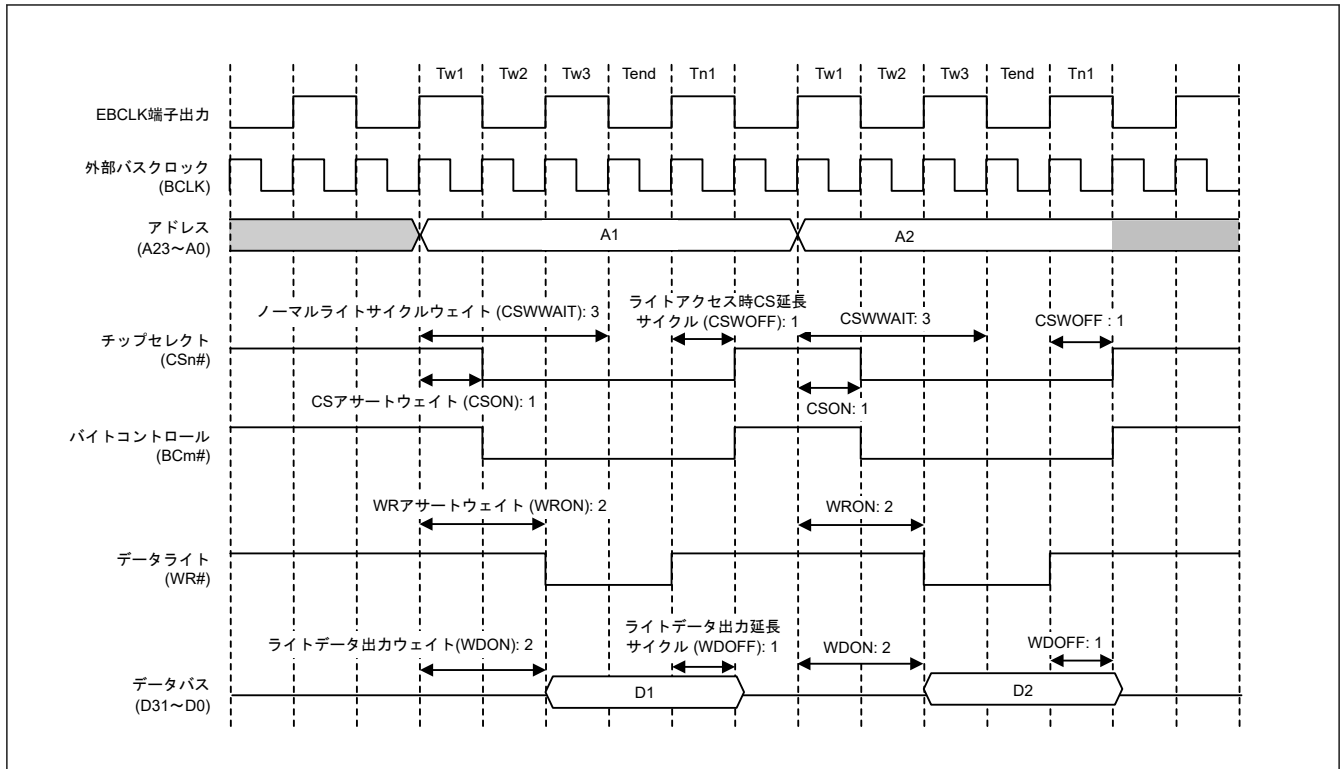
図 14.12 ノーマルライトアクセスの動作例 (EBCLK 端子出力選択ビットで BCLK の 2 分周を設定した場合) (n = 0~7, m = 0~3)
