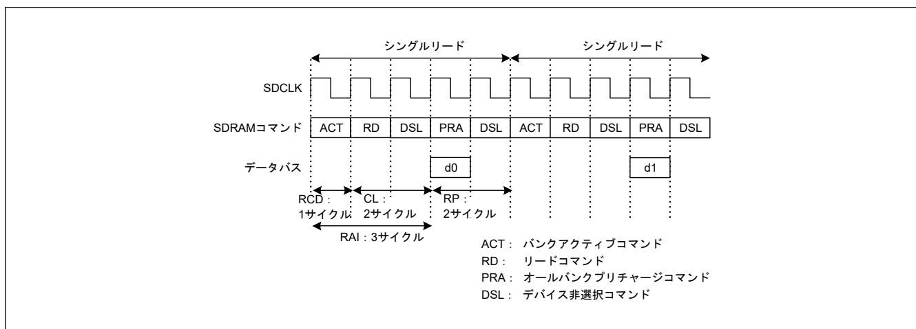
図 14.52 シングルリードタイミング例 (1)
