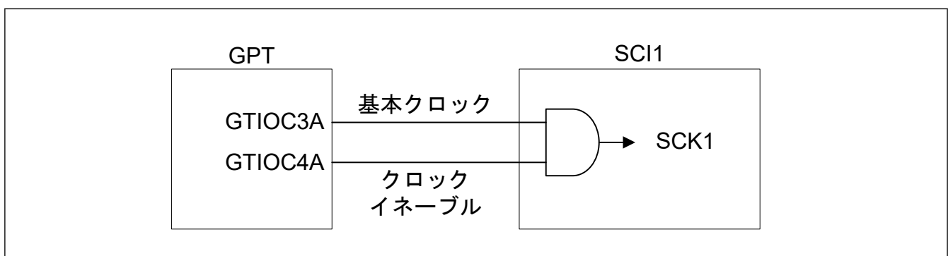
図 31.4 GPT と SCI の接続例
