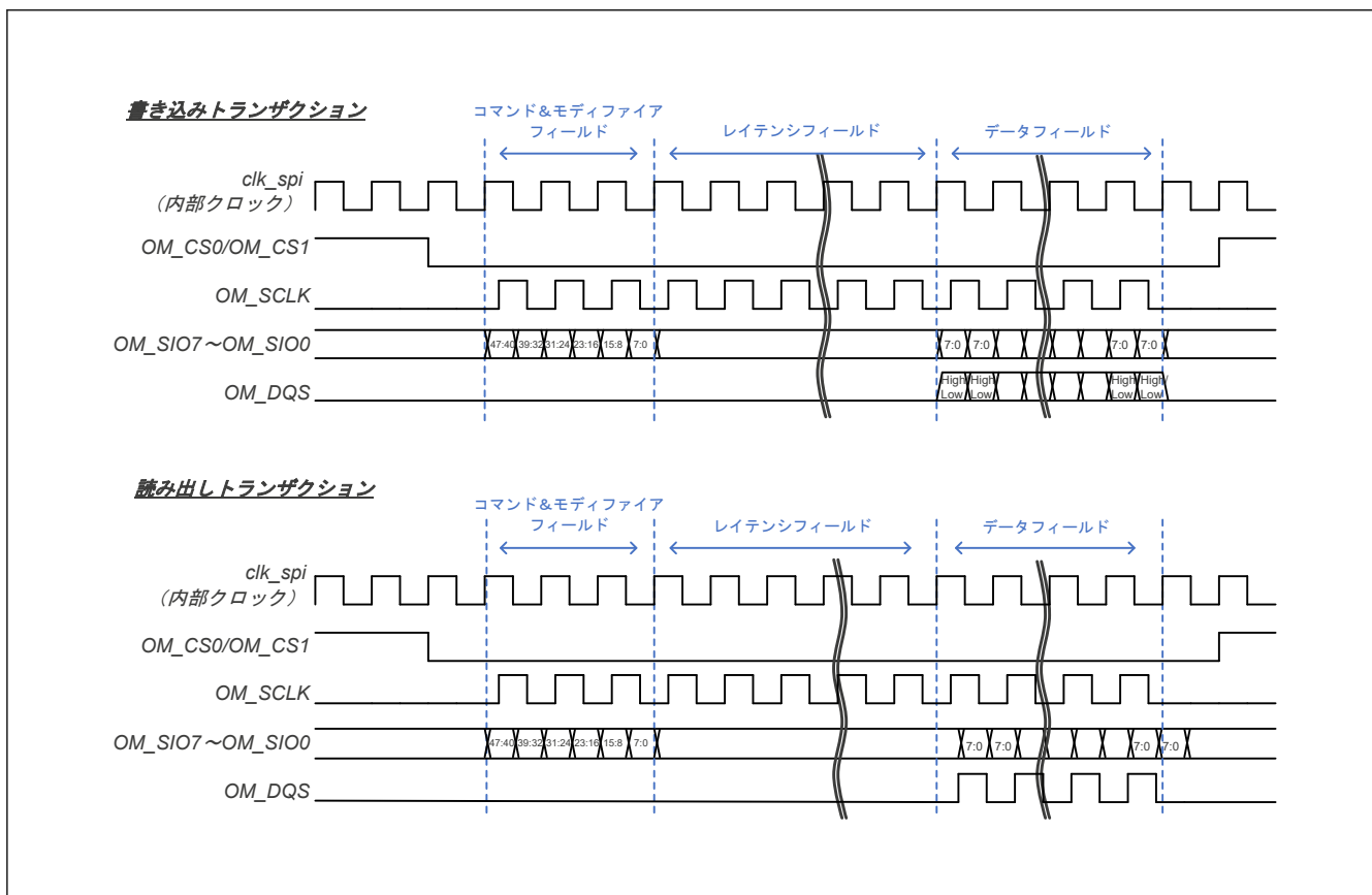
図 37.7 8D-8D-8D プロファイル 2.0 のタイミングチャート
