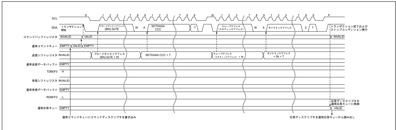
図 33.15 ダイナミックアドレス配置手順 (SETDASA CCC) タイミング
