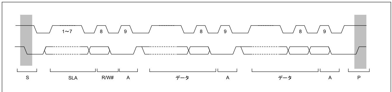
図 33.70 I 2 C バスタイミング (SLA = 7 ビットの場合)
