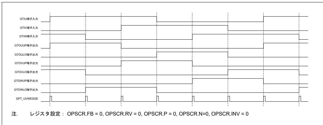
図 21.63 GPT OPS レベル出力動作例 (正転)
