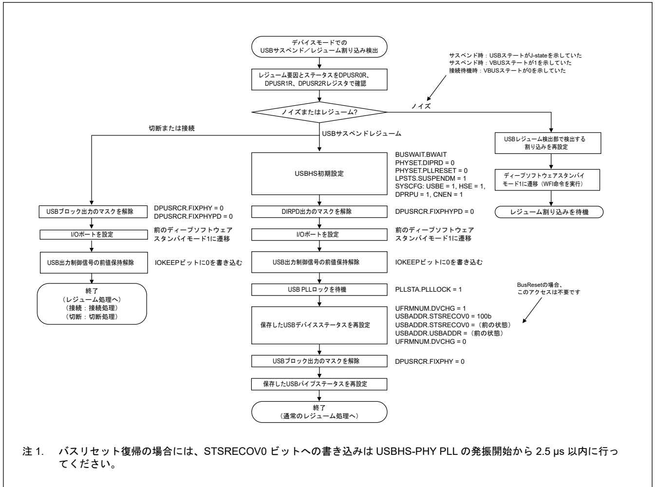
図 30.25 デバイスコントローラとしてディープソフトウェアスタンバイモード 1 を解除する場合の USBHS 設定フロー (1)
