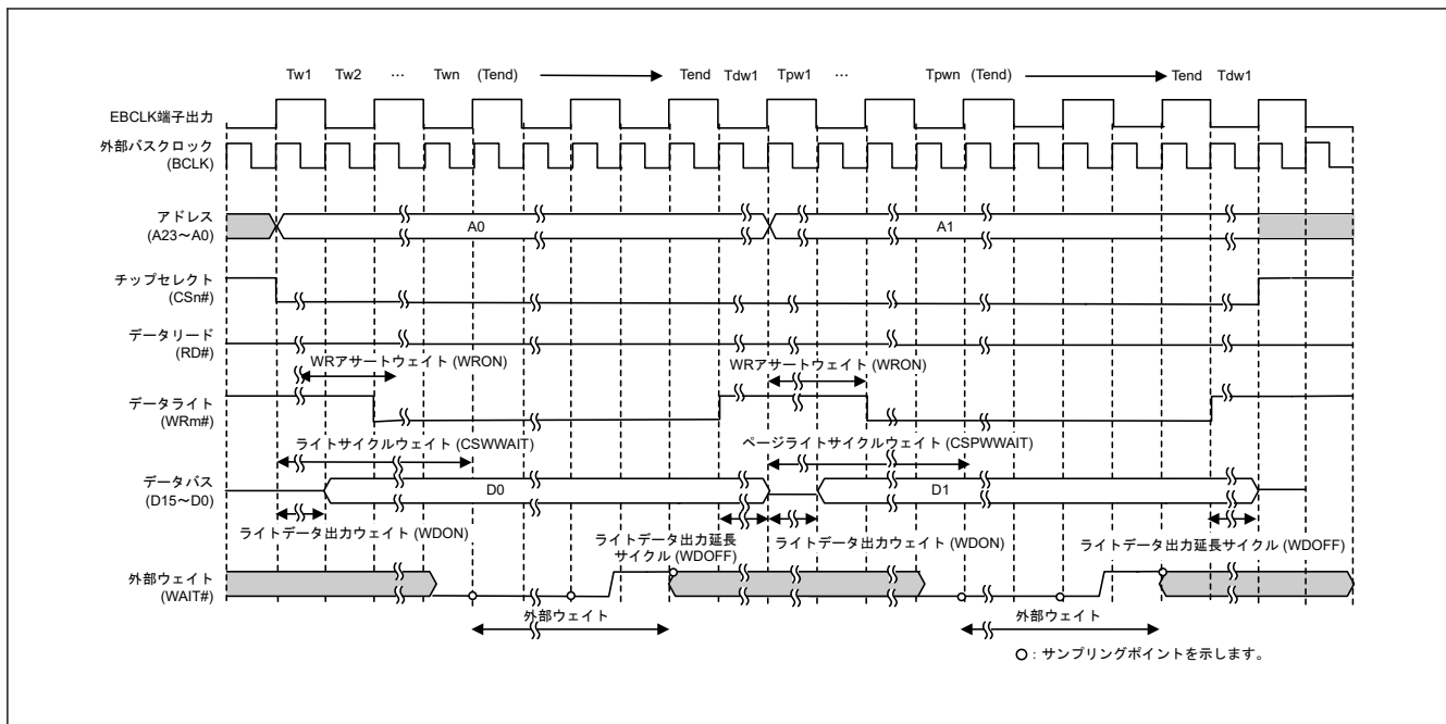
図 14.27 外部ウェイトタイミング例 (バイトストローブモード時の 16 ビットバス空間に対するページライトアクセス、EBCLK 端子出力選択ビットで BCLK の 2 分周を選択した場合) (n = 0~7, m = 0, 1)
