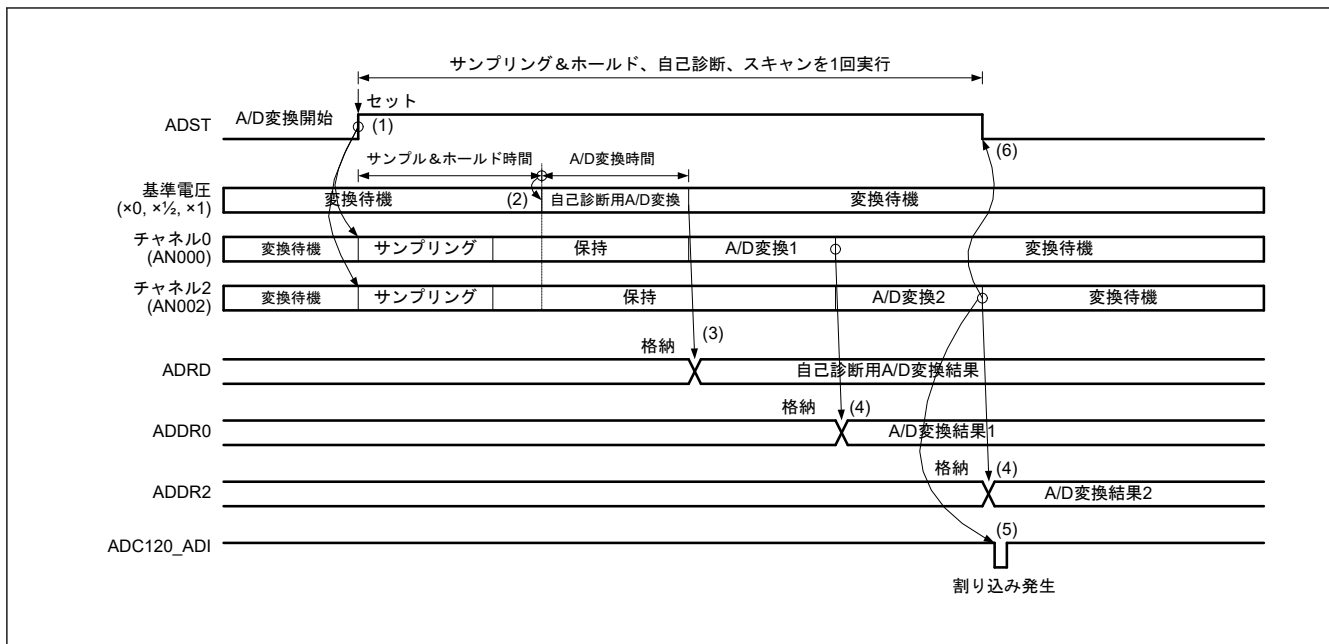
図 45.12 シングルスキャンモードの動作例 (チャンネル専用サンプル&ホールド回路使用、AN000~AN002 選択 + 自己診断、連続サンプリング無効)
