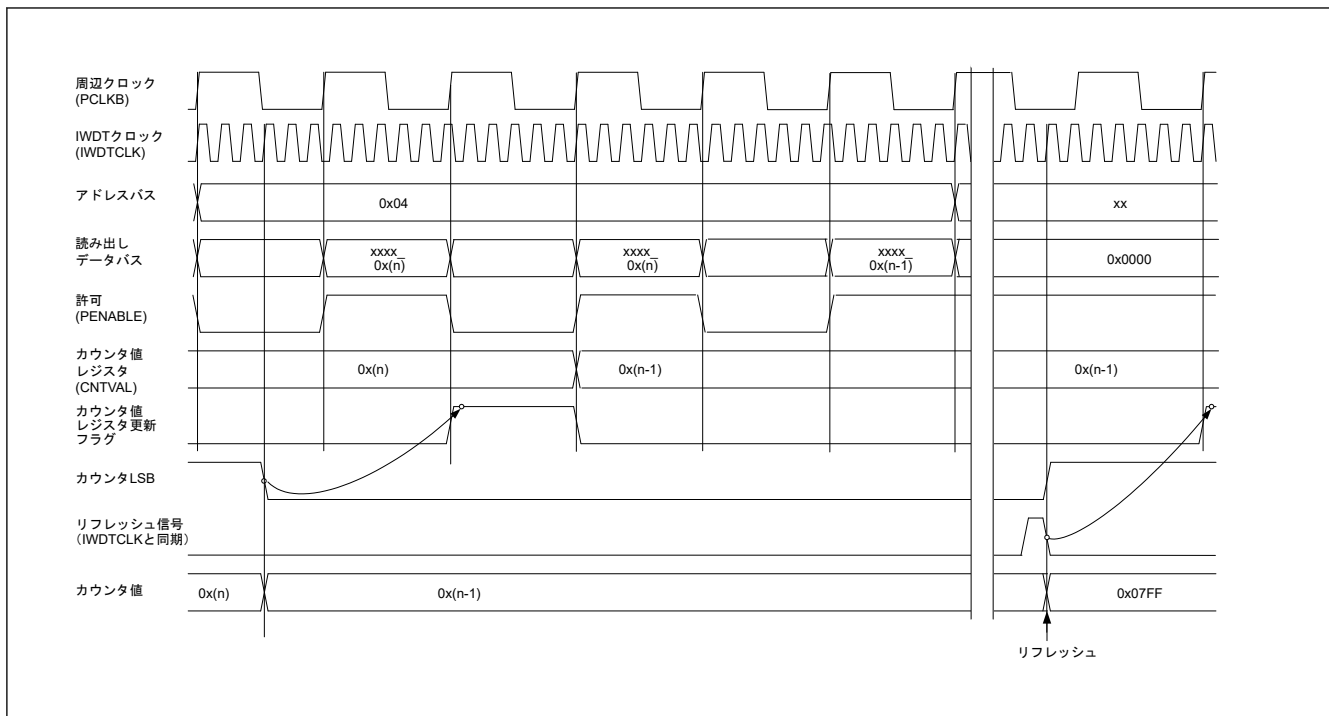
図 26.9 IWDT カウンタ値の読み出し処理 (IWDTCR.CKS[3:0] = 0010b、IWDTCR.TOPS[1:0] = 11b の場合)
