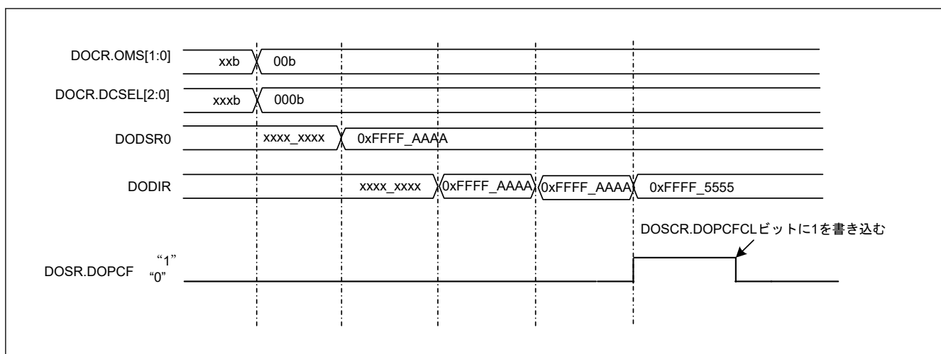
図 49.2 データ比較モードの動作例 (検出条件 : 不一致)
