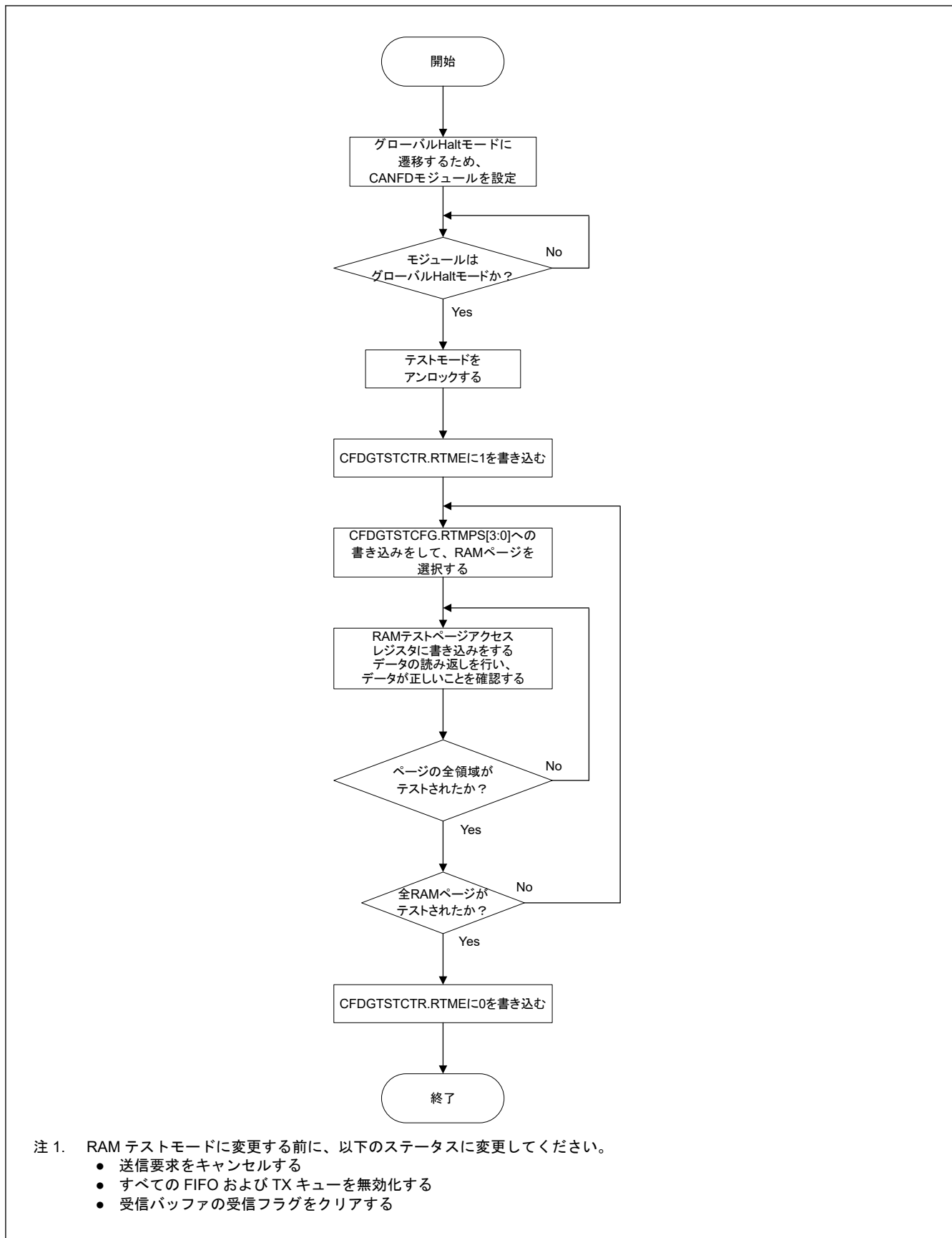
図 34.53 RAM テストモードのソフトウェアフロー
