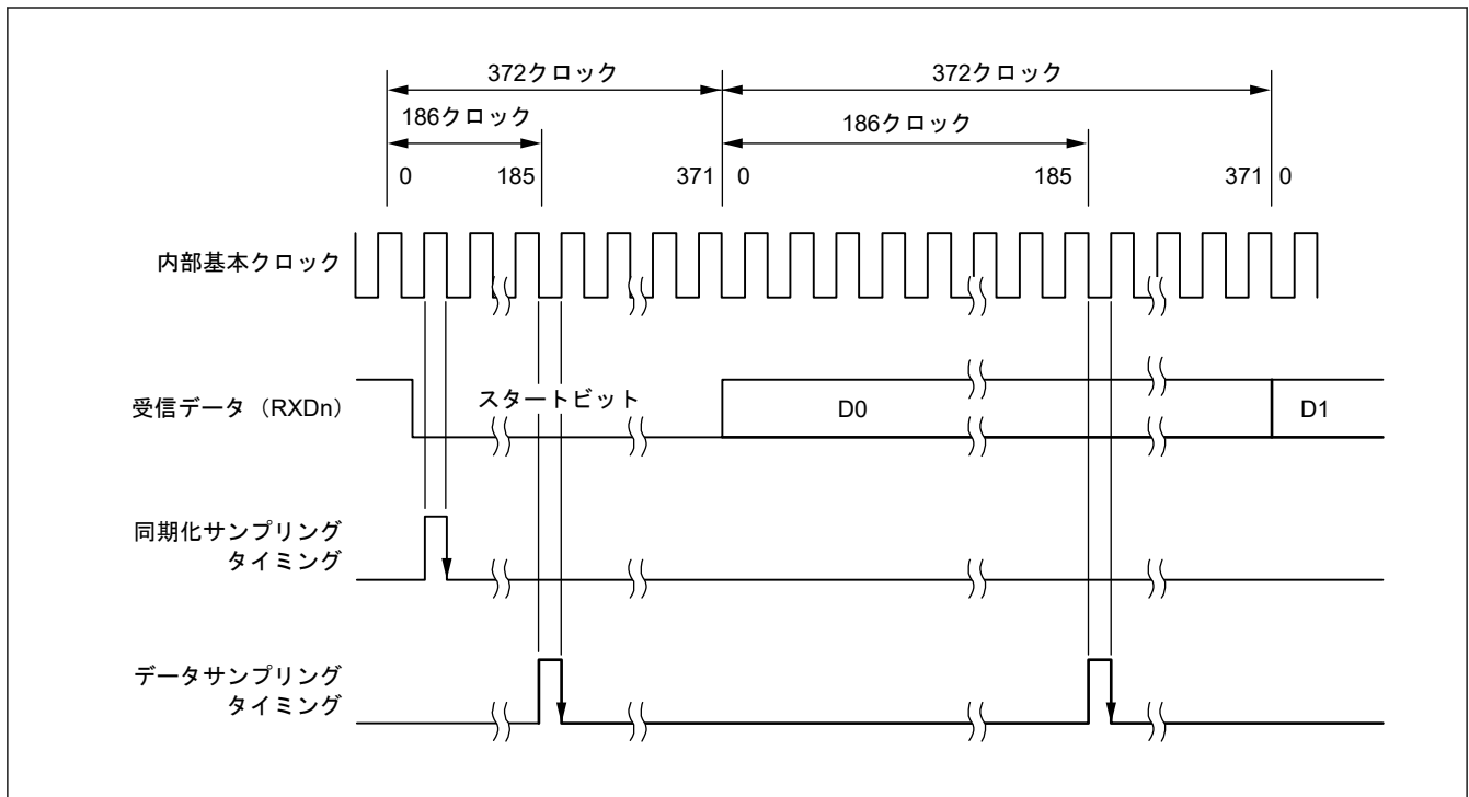
図 31.78 スマートカードインタフェースモードにおける受信データのサンプリングタイミング (ビットレートが 372 倍のクロック周波数の場合)
