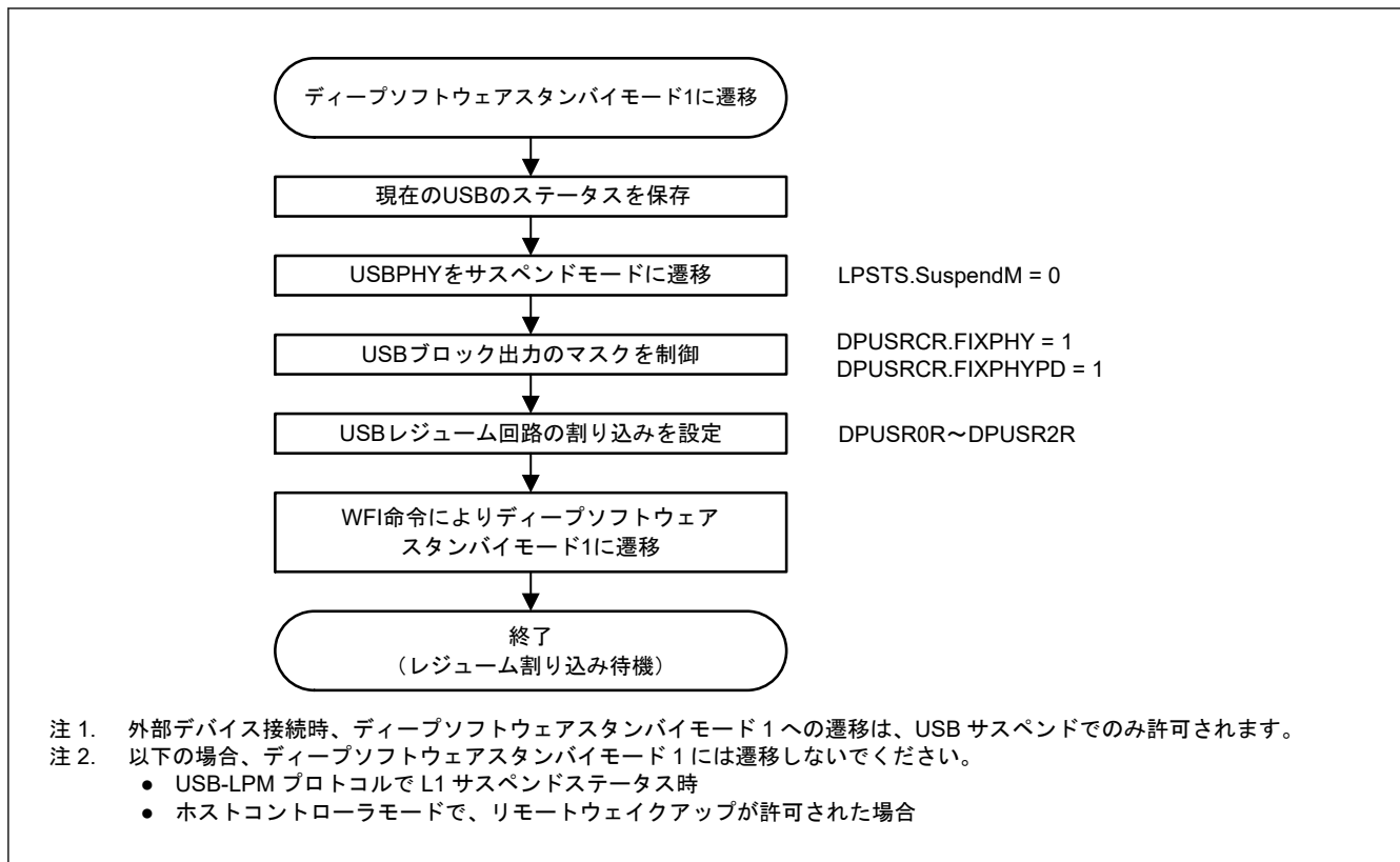
図 30.22 ホストコントローラまたはデバイスコントローラとしてディープソフトウェアスタンバイモード1へ遷移する場合の USBHS 設定フロー
