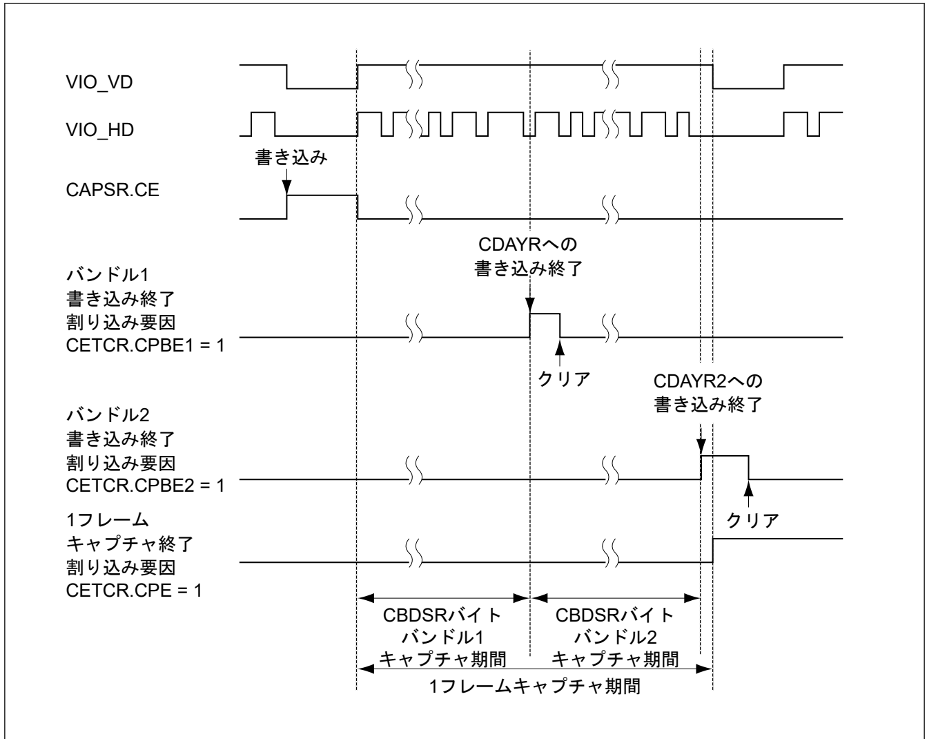
図 53.43 書き込み終了割り込みのタイミング (データイネーブル取り込み時)
