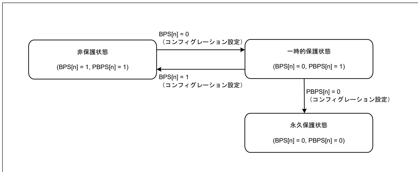
図 52.37 BPS[n]ビットおよびPBPS[n]ビットによるフラッシュシーケンサの状態遷移
