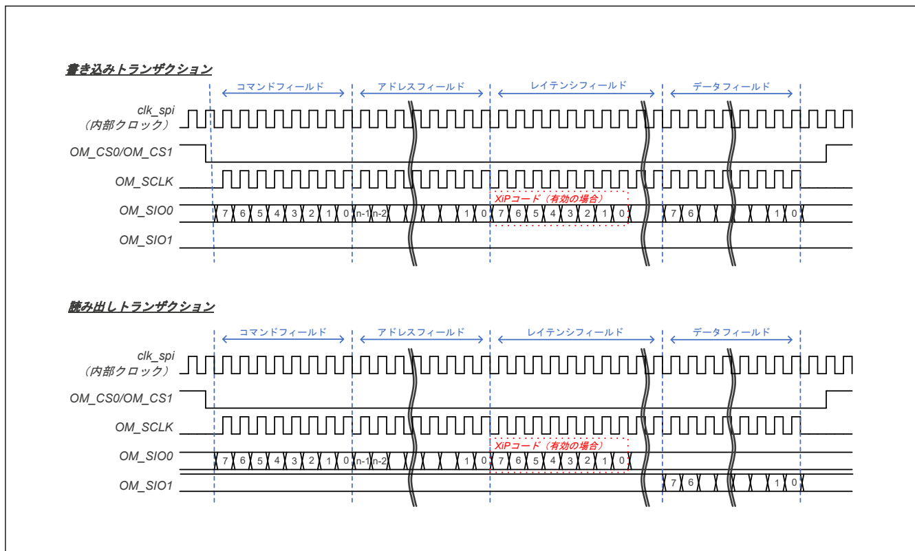
図 37.3 1S-1S-1S のタイミングチャート
