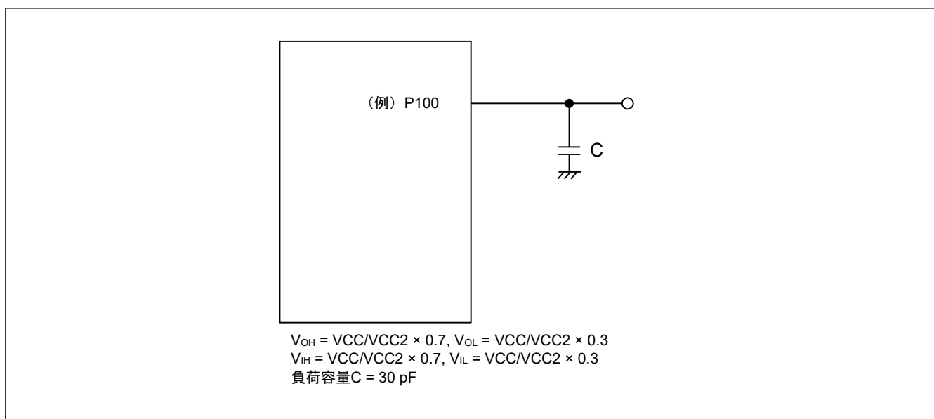
図 55.1 入出力タイミング計測条件
