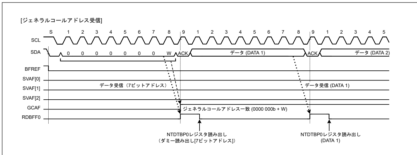
図 33.85 ジェネラルコールアドレス受信時に GCAF フラグが 1 になるタイミング
