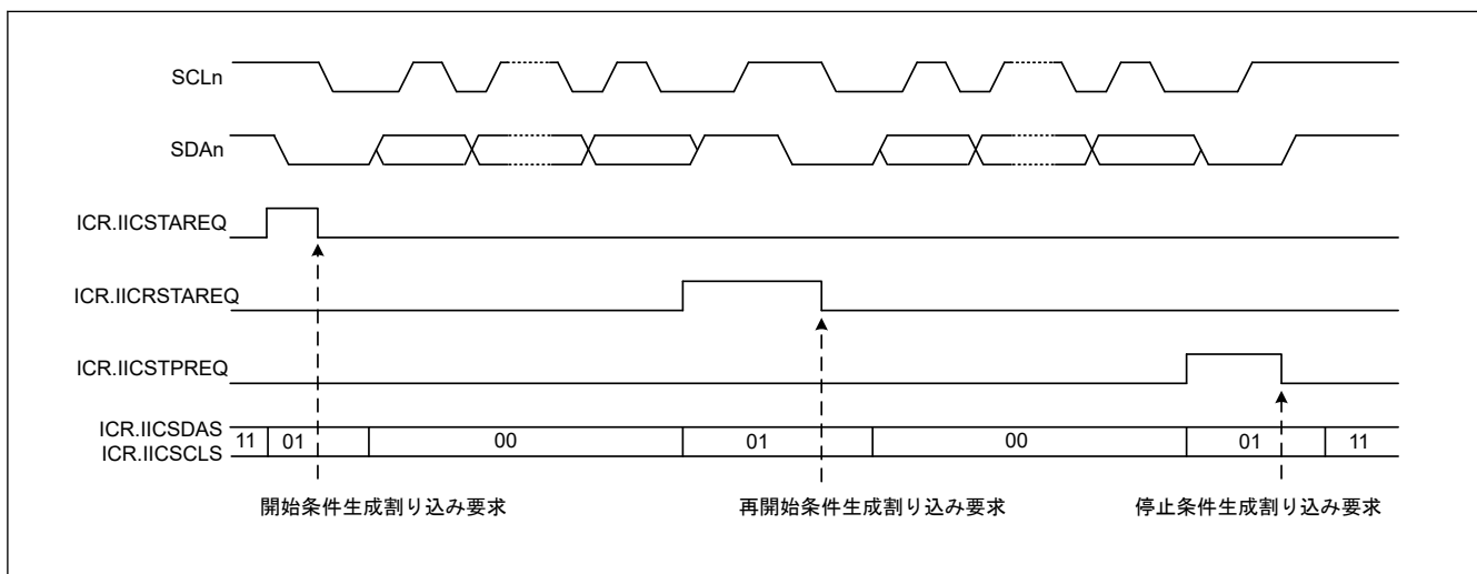
図 31.88 開始条件、再開条件、停止条件生成の動作タイミング
