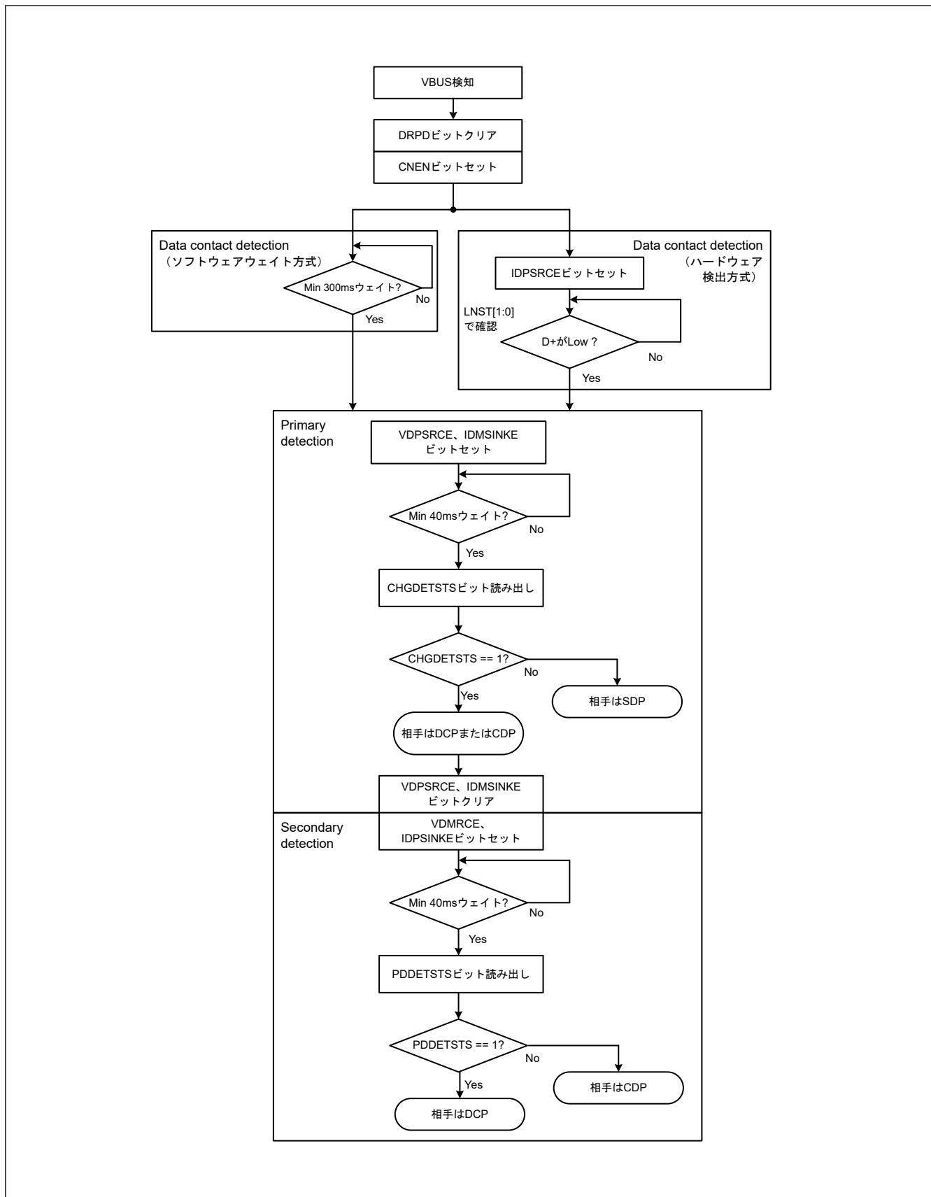
図 30.19 Portable Device としての処理フロー
