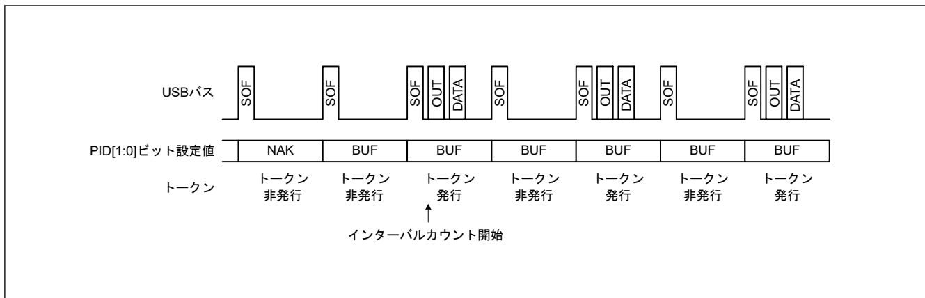
図 30.13 IITV[2:0] = 1 の場合におけるトークン発行の有無
