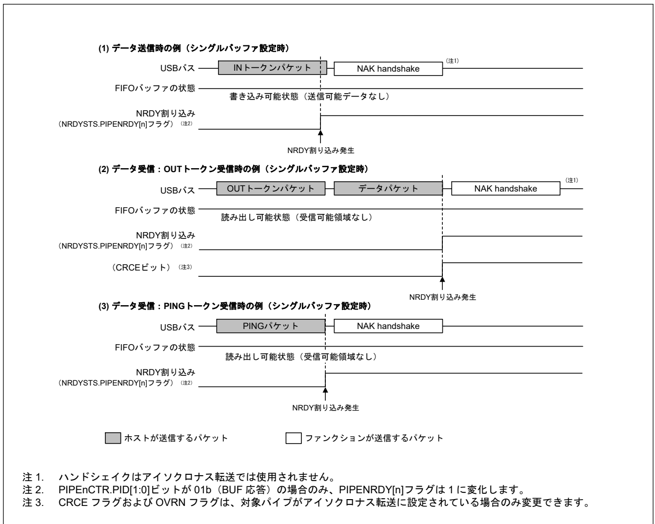
図 30.6 デバイスコントローラモード時の NRDY 割り込み発生タイミング
