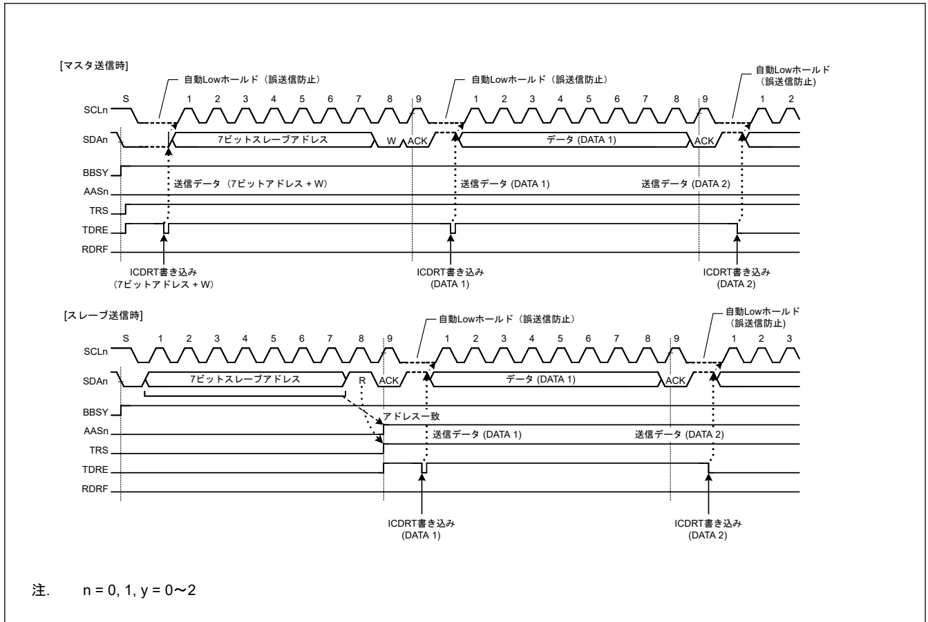
図 32.38 送信モード時の自動 Low ホールド動作
