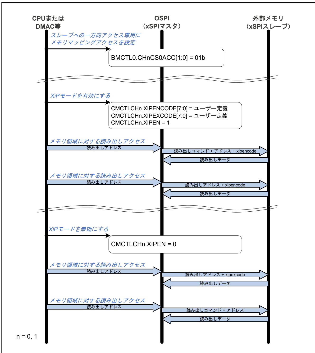
図 37.30 XiP モード有効/無効のフロー
