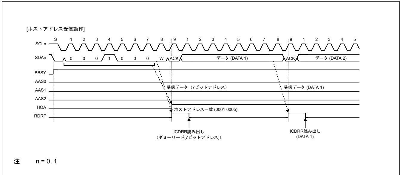
図 32.29 ホストアドレス受信時に HOA フラグが 1 になるタイミング
