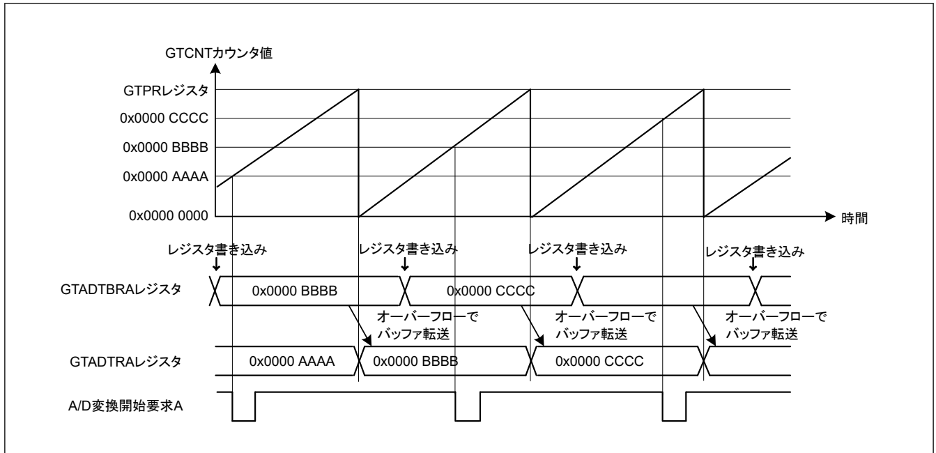
図 21.18 GTADTRA および GTADTRB レジスタのバッファ動作例 (のこぎり波でアップカウント、アップカウントで A/D 変換開始要求発生の場合)
