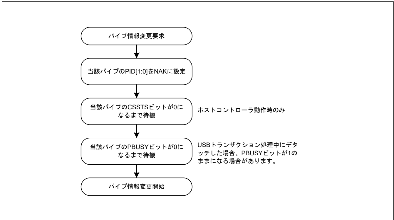
図 30.10 USB 通信が許可状態で PID[1:0]ビットが 01b (BUF 応答) のときのパイプ情報変更手順
