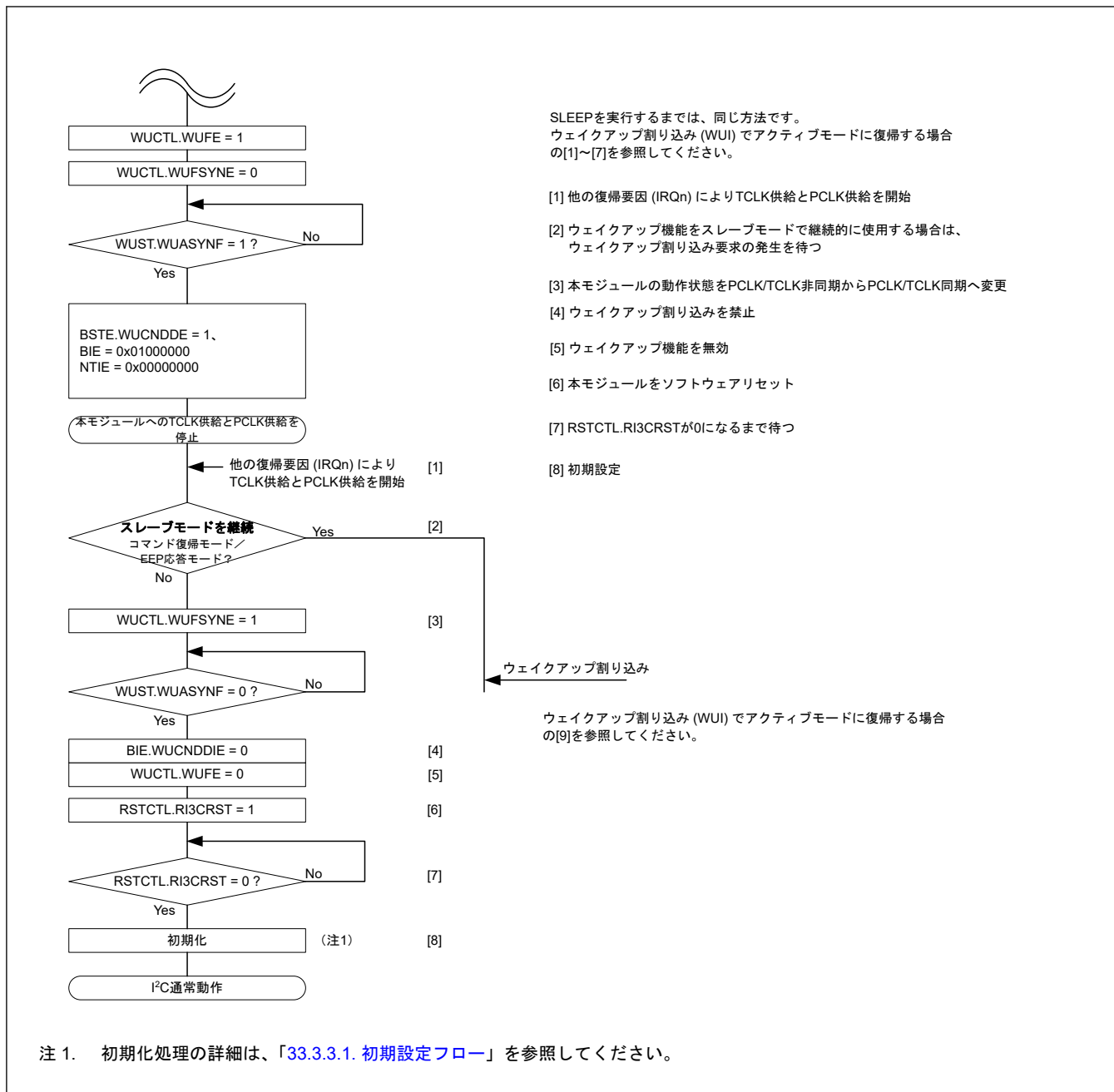
図 33.132 コマンドリカバリモードと EEP 応答モードの使用例 (他のリカバリ要因 (IRQ) によるウェイクアップリカバリの場合)
