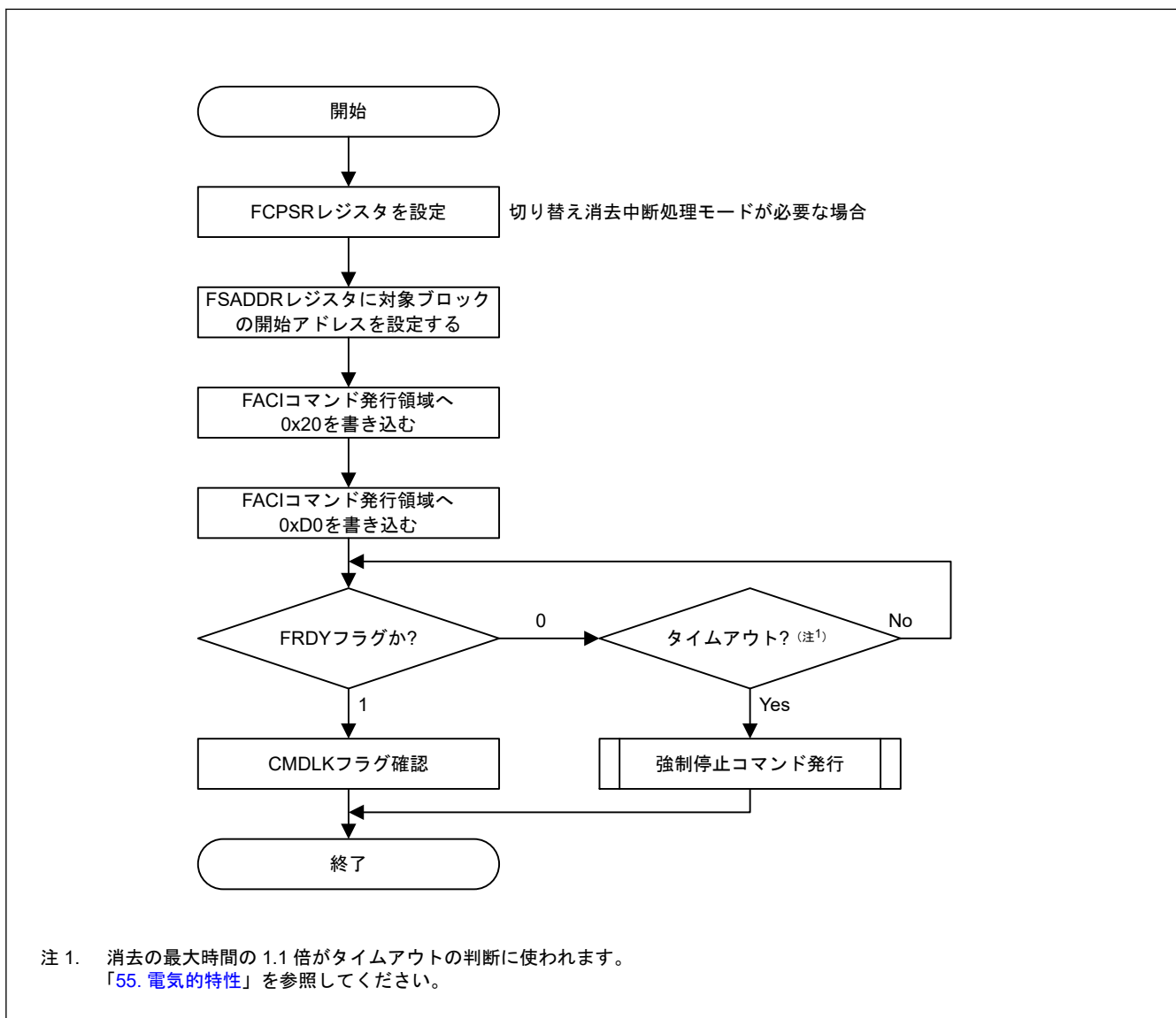
図 52.15 ブロックイレースコマンドの使用フロー
