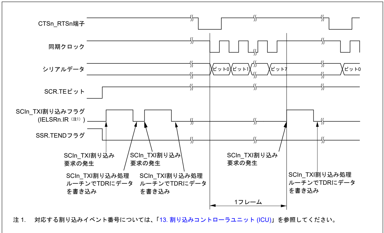
図 31.63 クロック同期式モードにおけるシリアル送信の動作例 (送信開始時に CTS 機能を使用する場合)
