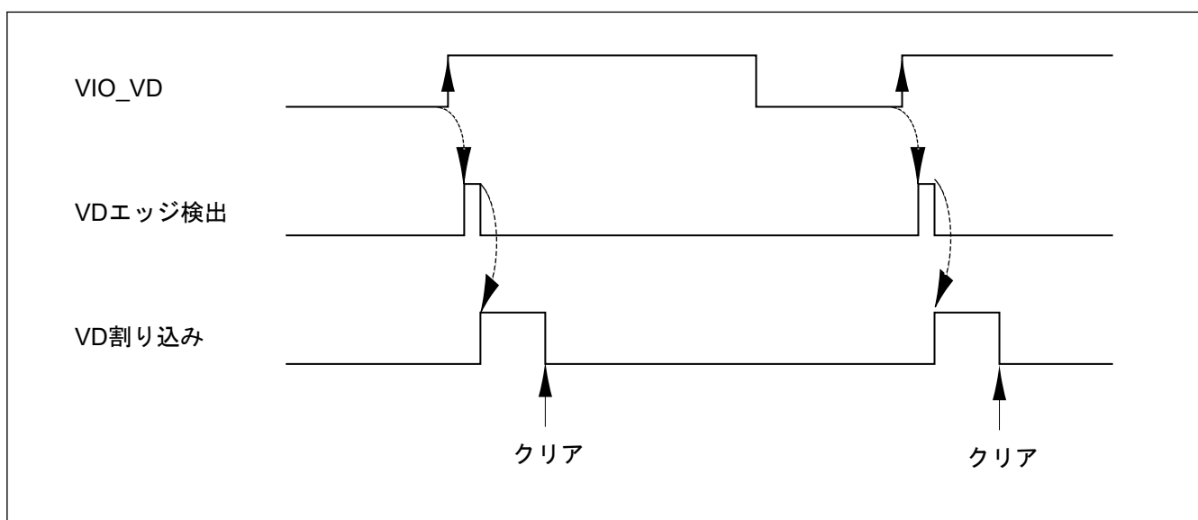
図 53.14 VD が正極性の場合の VIO_VD と VD 割り込みの関係(データイネーブル取り込みモードの場合)
