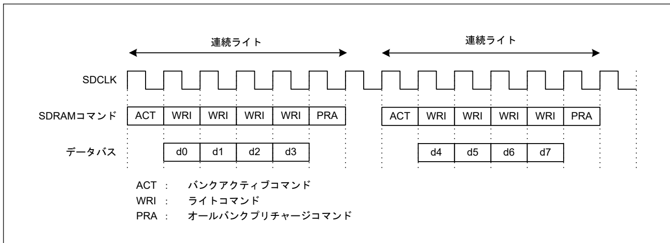
図 14.47 連続ライトのタイミング例 (SDAMOD.BE = 1、最も早いタイミングを設定したとき)
