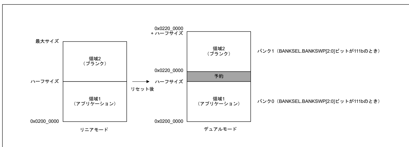
図 52.51 リニアモードでのデュアルモード用アプリケーションの書き込み
