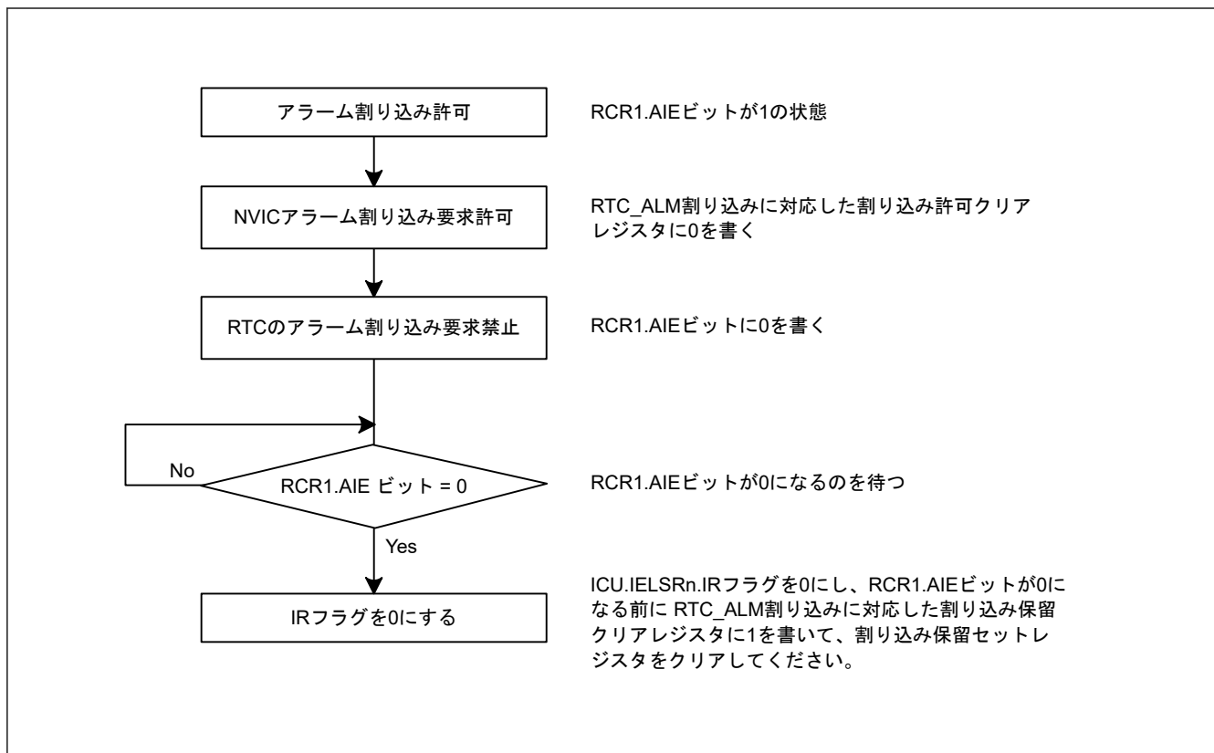
図 24.8 アラーム割り込み要求の禁止手順
