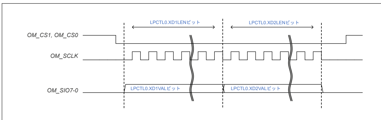
図 37.19 XiP 禁止パターン
