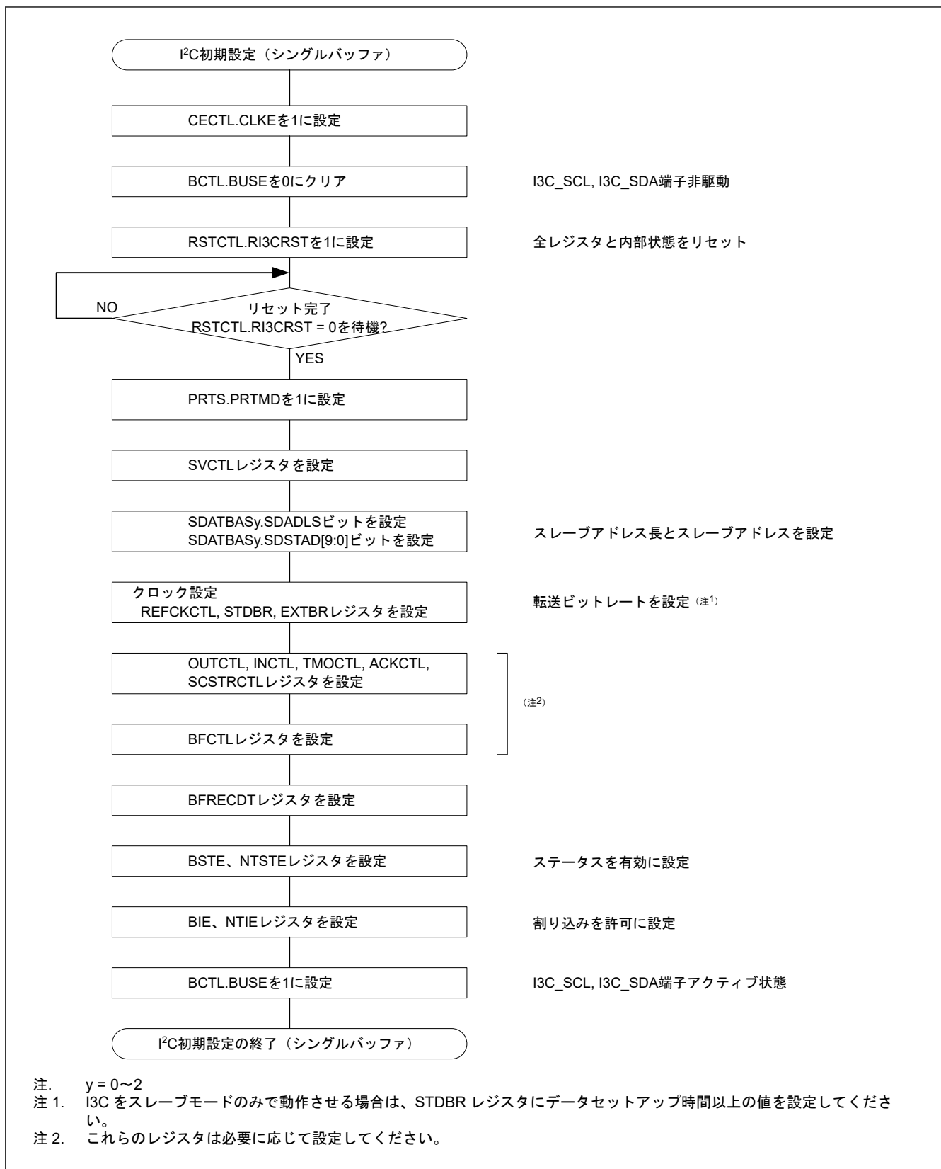
図 33.140 I²C 初期化フローチャート例 (シングルバッファ転送)
