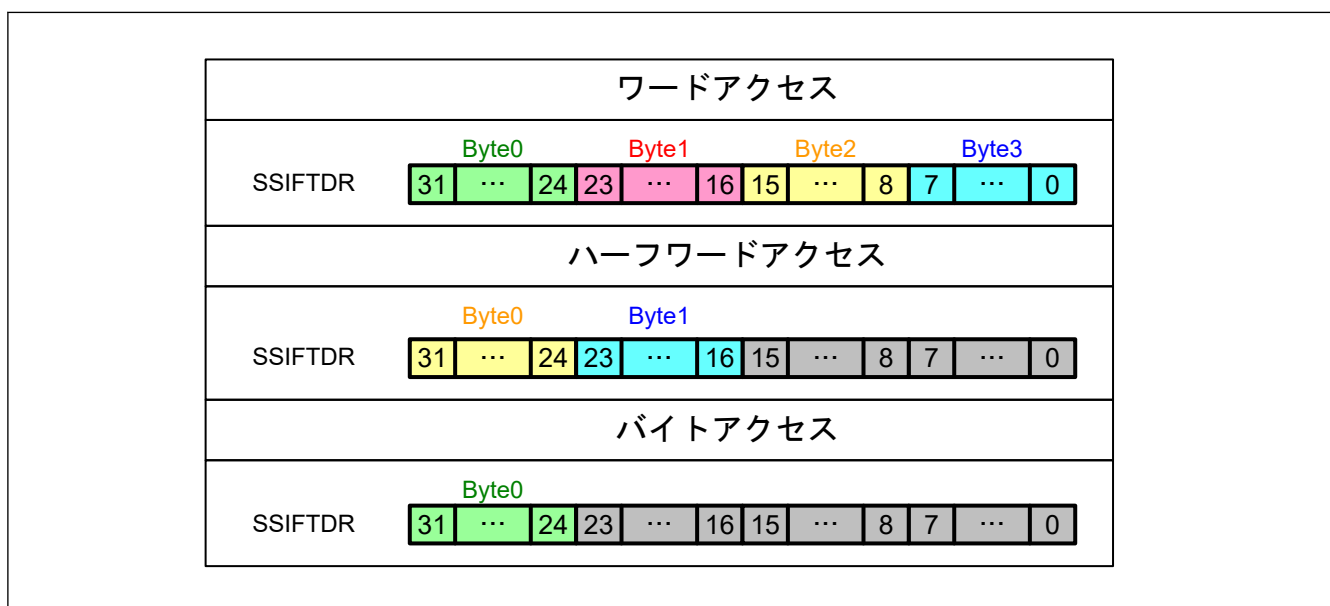
図 39.30 送信 FIFO データレジスタへのレジスタアクセスの例
