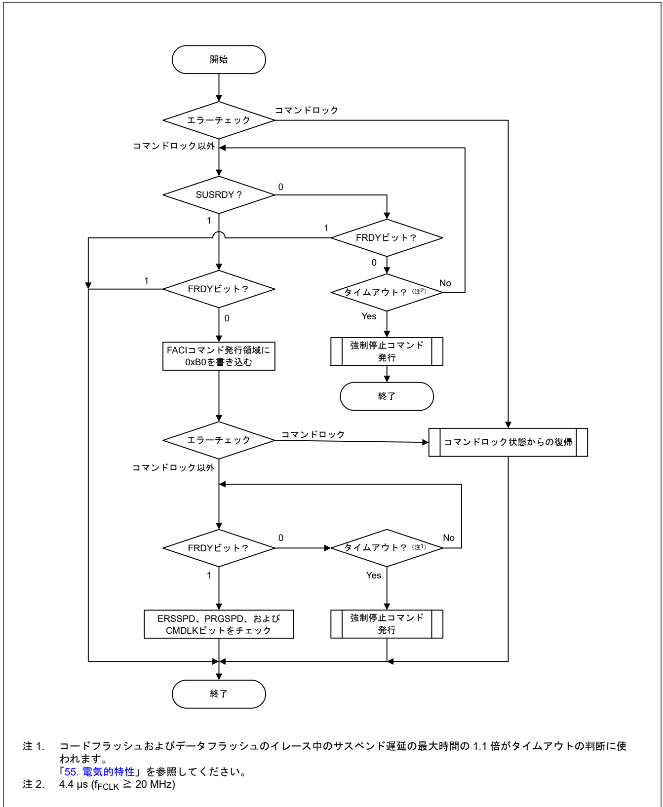
図 52.17 P/E サスペンドコマンドの使用フロー
