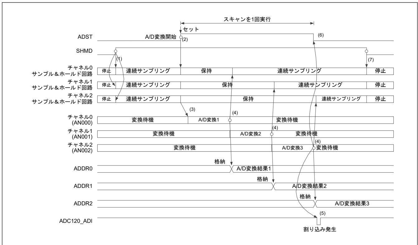
図 45.10 シングルスキャンモードの動作例（チャンネル専用サンプル&ホールド回路使用、AN000～AN002 選択、連続サンプリング有効）
