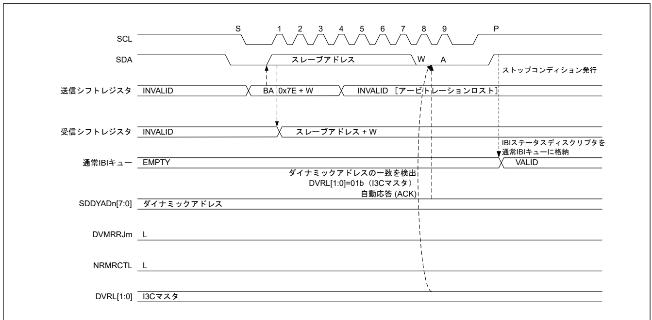
図 33.105 バス権要求 : ACK
