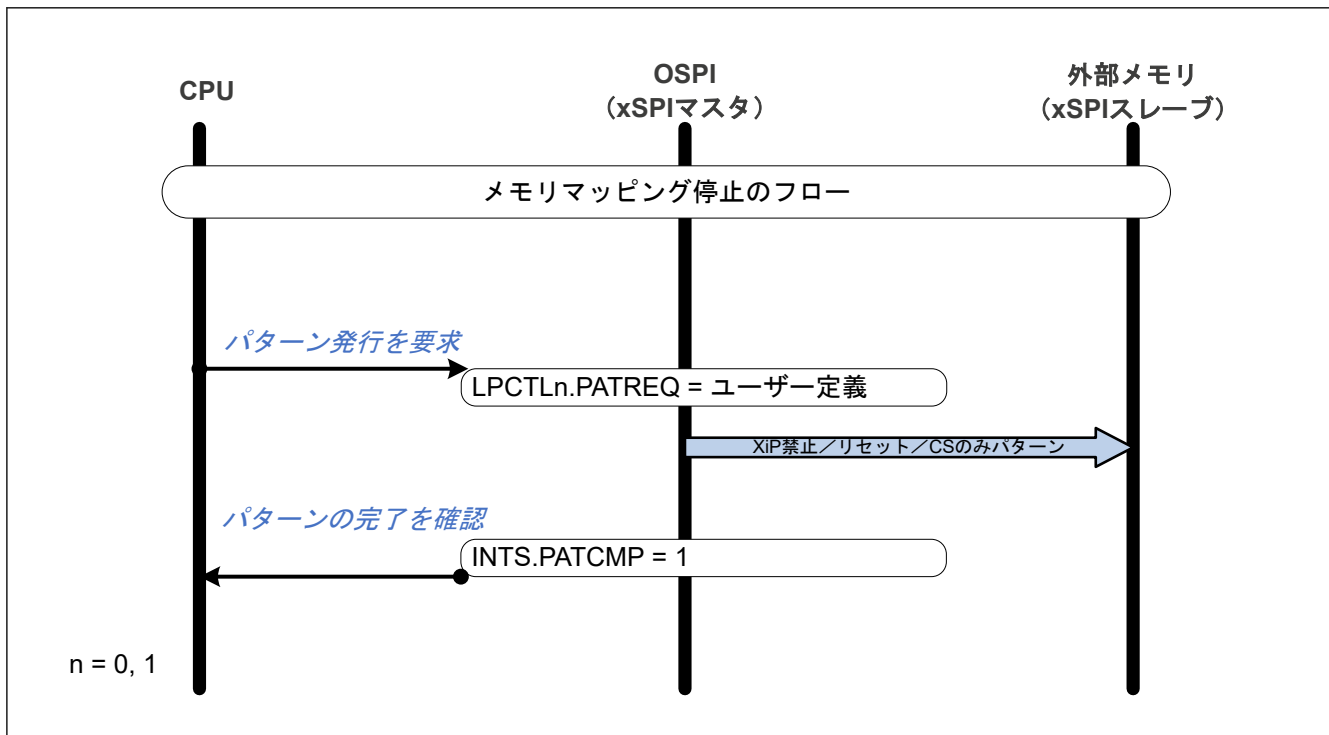
図 37.29 パターン要求のフロー
