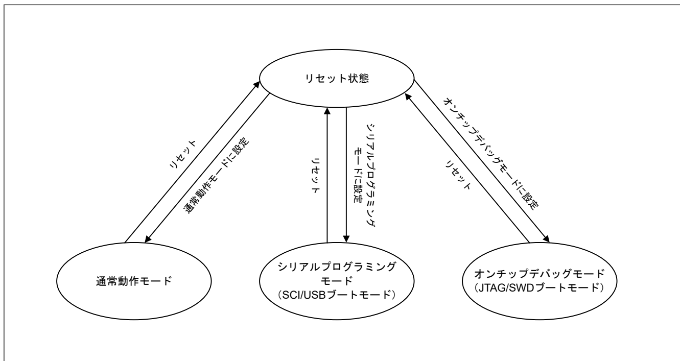
図 52.6 フラッシュメモリに関するモード遷移図
