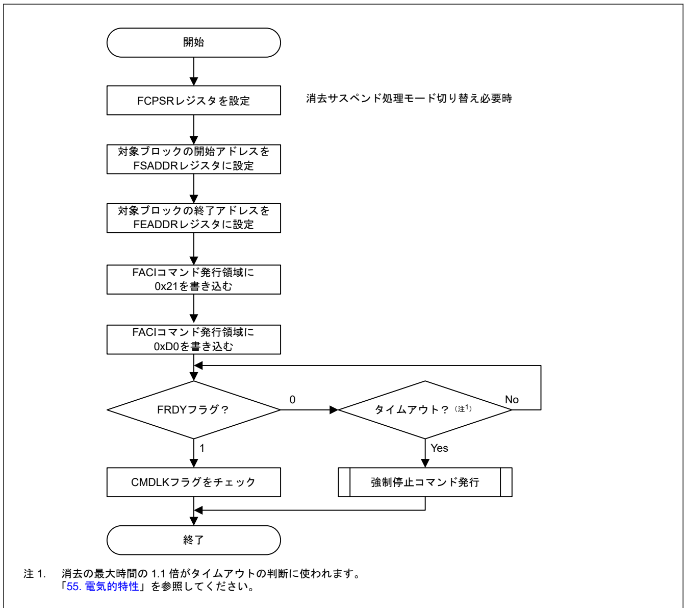
図 52.16 マルチブロックコマンドの使用フロー
