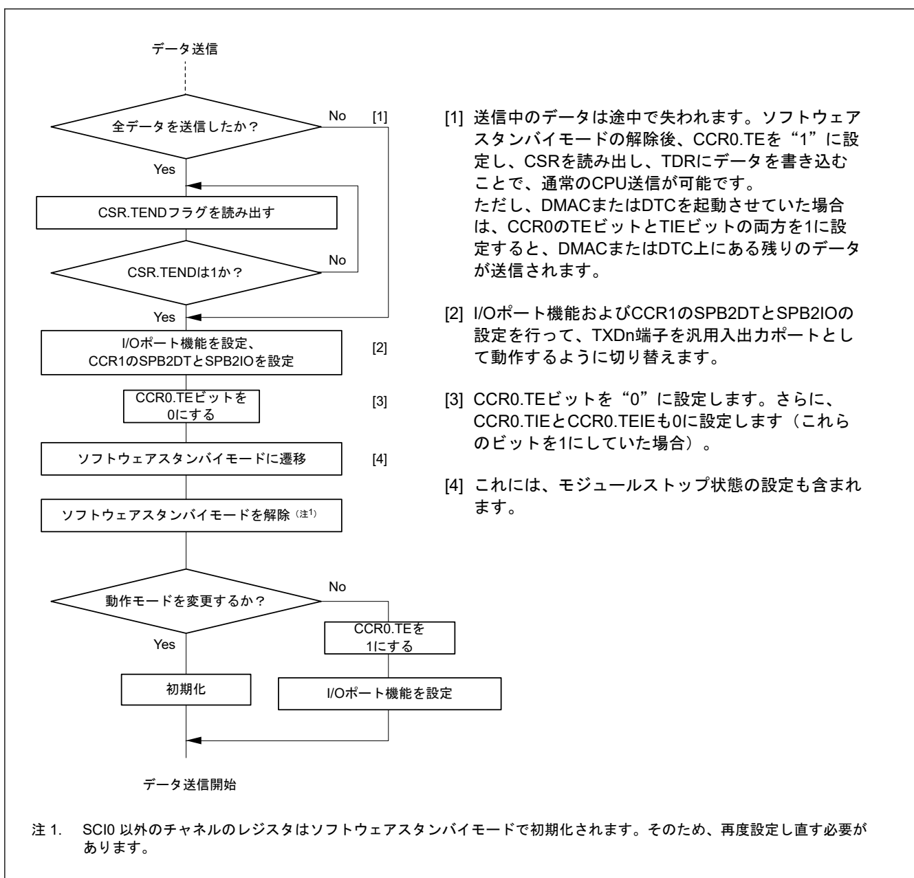
図 31.117 送信時にソフトウェアスタンバイモードに遷移する場合のフローチャート例
