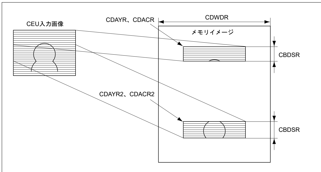
図 53.41 バンドル書き込みメモリ格納イメージ
