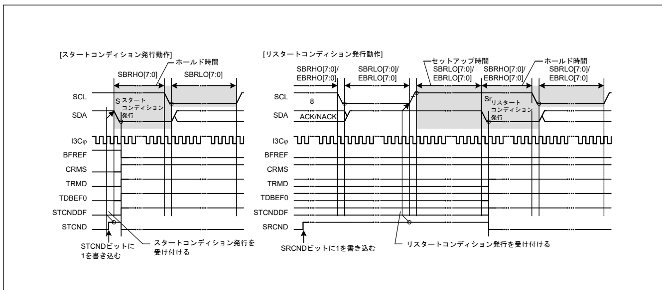
図 33.79 スタートコンディション/繰り返しのスタートコンディション発行動作タイミング (STCND、SRCND ビット)
