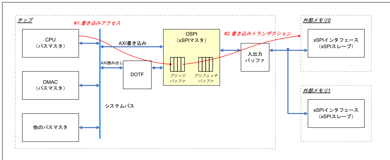
図 37.12 メモリ領域に対する書き込みアクセス
