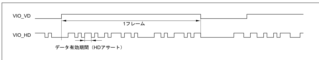
図 53.5 フレームのタイミング (データイネーブル取り込みの場合)
