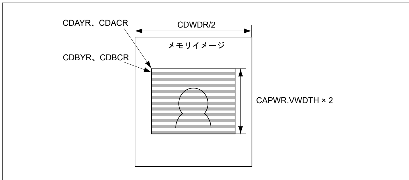
図 53.29 インターレース入力のフレームイメージメモリ格納イメージ
