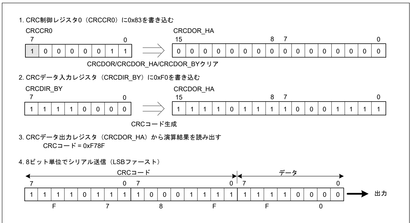
図 41.2 LSB ファーストのデータ送信
