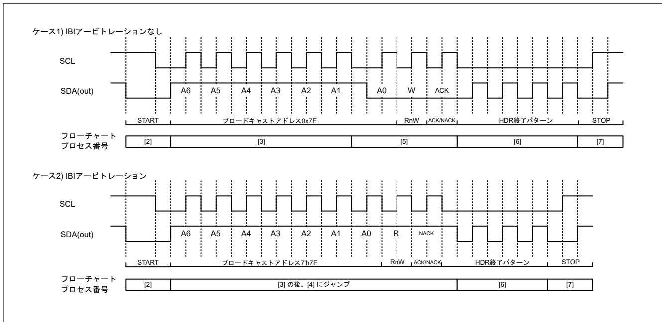
図 33.125 I3C マスタの I3C エスカレーション処理タイミングチャート
