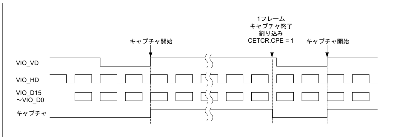
図 53.46 CPE 発生タイミング
