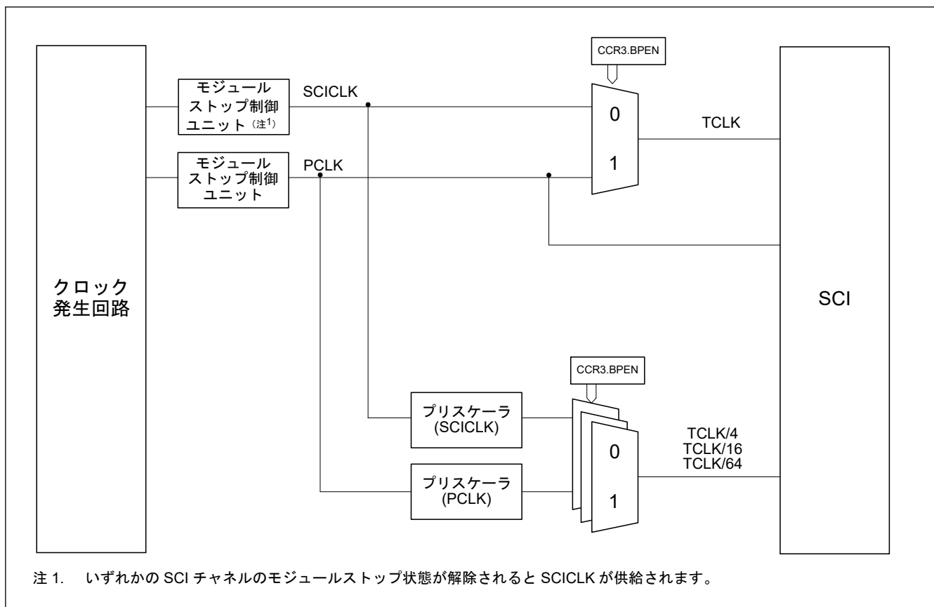
図 31.2 クロックソースセレクタのブロック図
