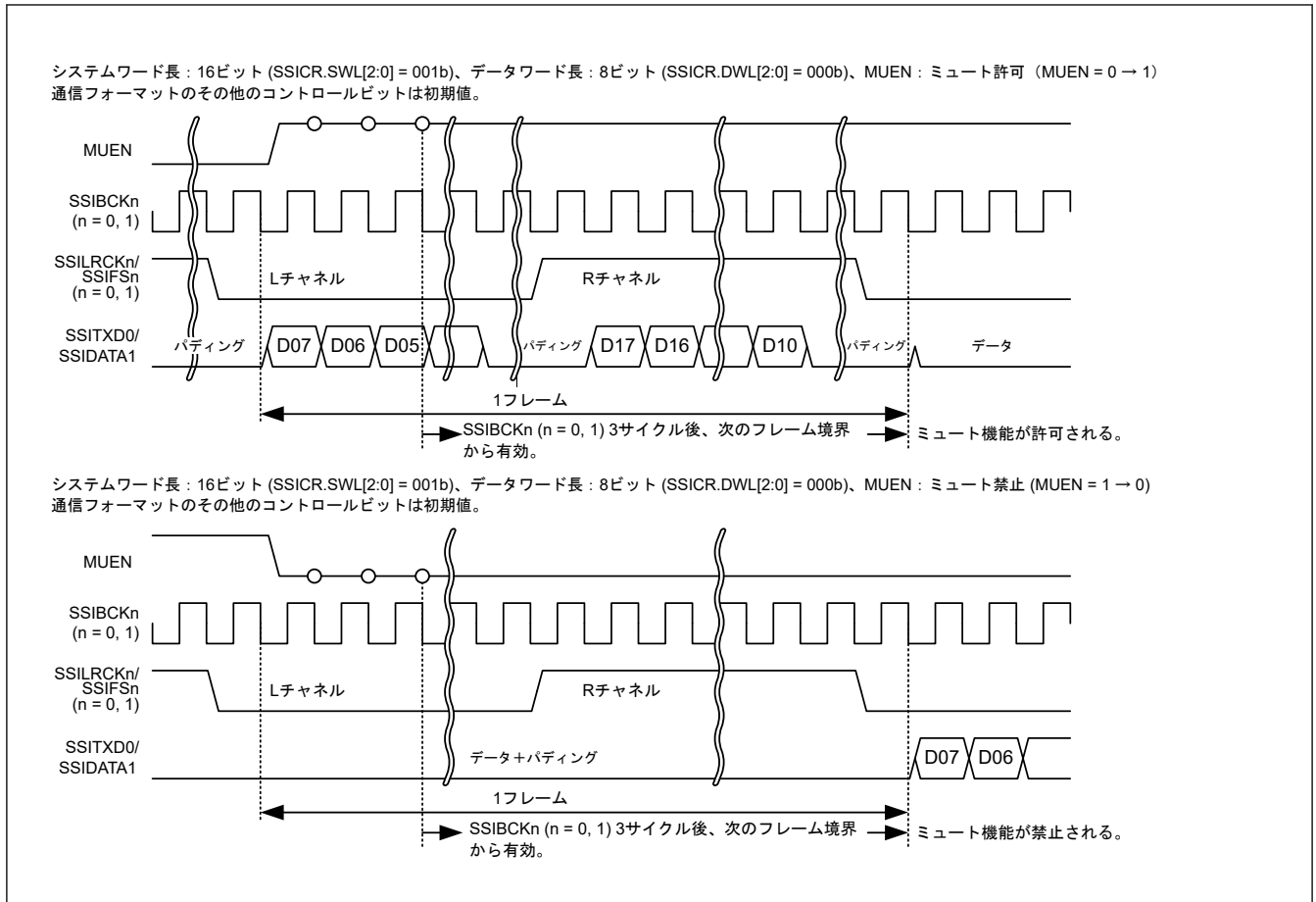
図 39.5 ミュート機能設定時のデータ送信
