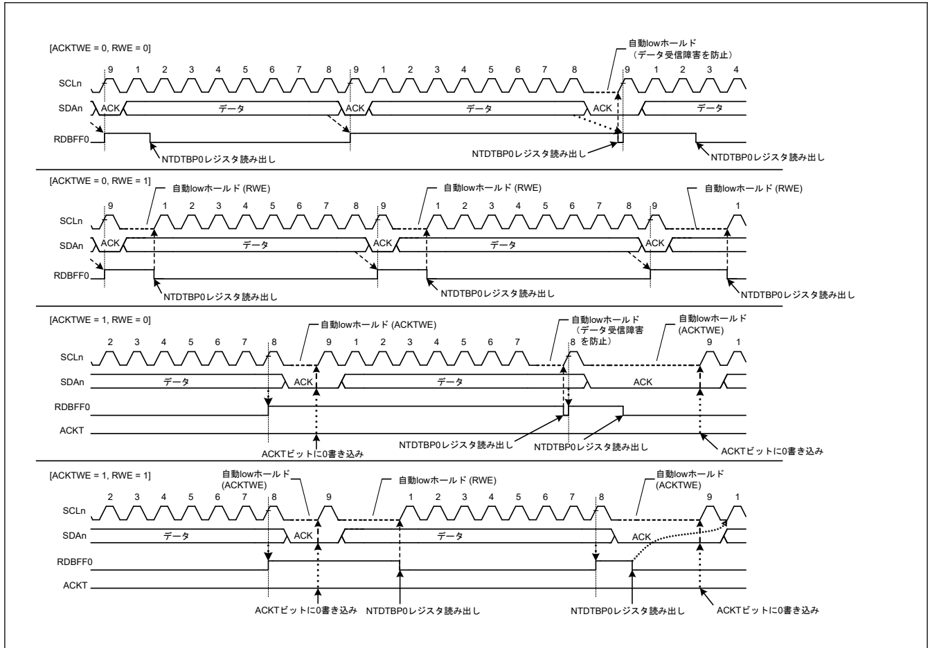
図 33.95 受信モード時の自動 Low ホールド動作 (ACKTWE および RWE ビットを使用)
