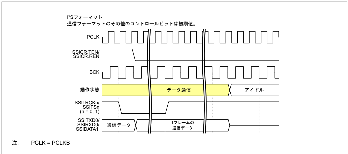
図 39.48 データ通信からの停止 (パディングビットなし)
