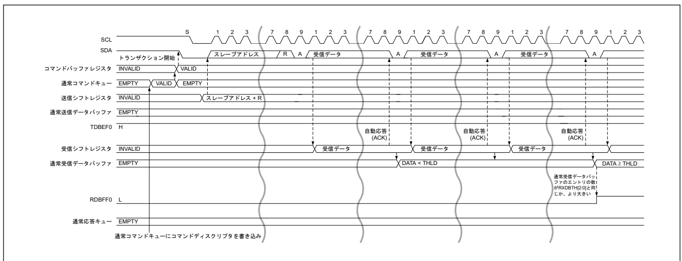
図 33.22 レガシー I2C メッセージデータ読み出し転送タイミング (1/2)
