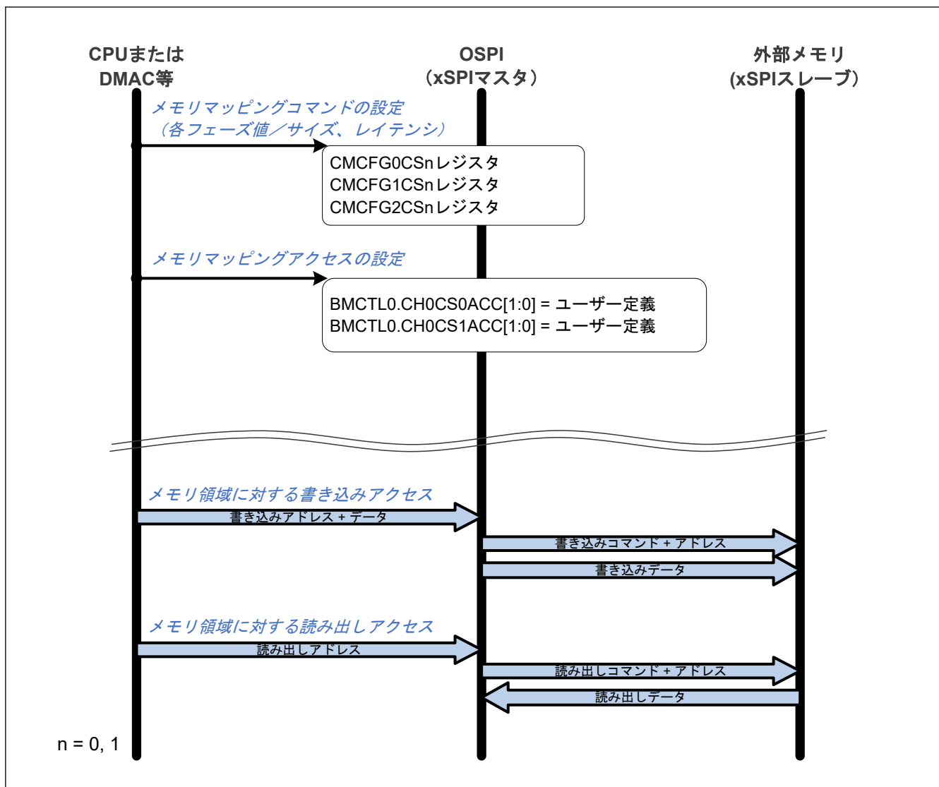
図 37.27 メモリマッピングのフロー
