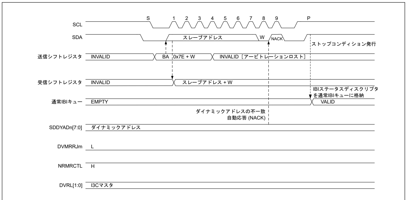
図 33.106 バス権要求 : NACK (DAT.DVDYAD[7:0]ビットが一致しない) かつ NRMRCTL が 1 の場合
