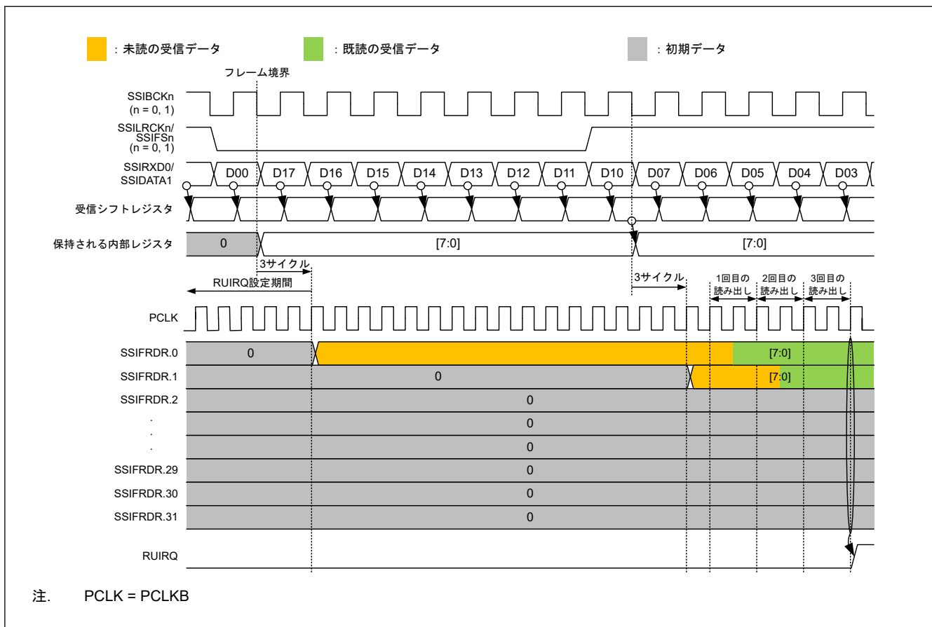
図 39.17 RUIRQ 設定タイミング
