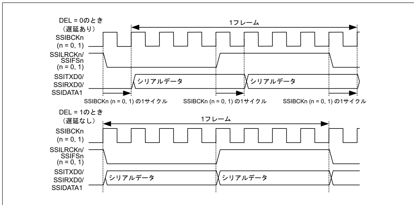
図 39.7 シリアルデータにおける遅延の設定
