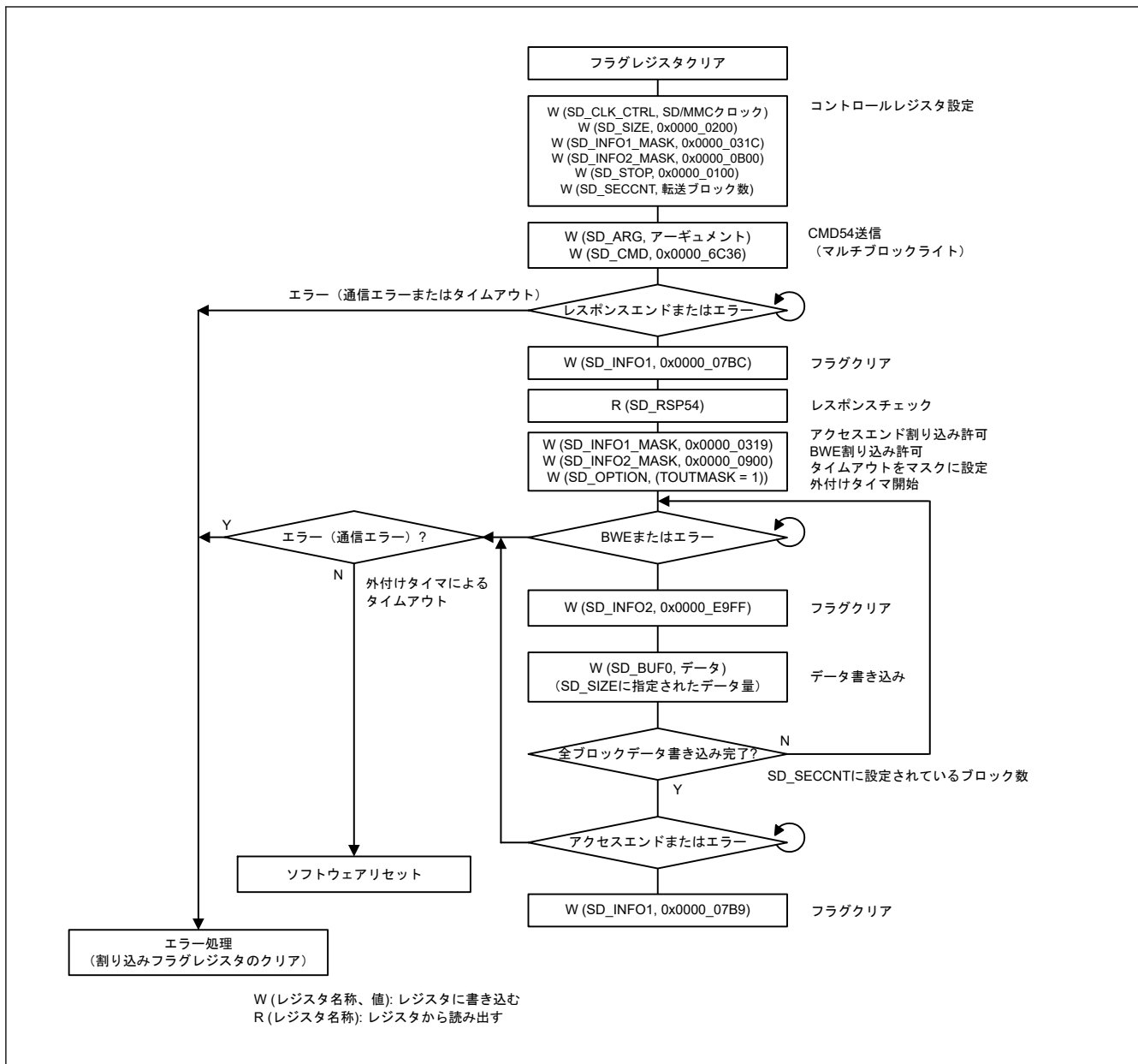
図 40.15 外付けタイマによるマルチブロックライト動作の例
