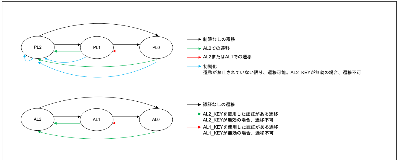
図 43.8 PL/AL 状態と遷移
