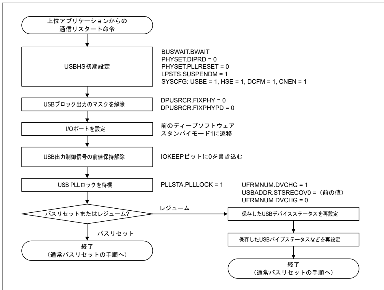
図 30.24 ホストコントローラとしてディープソフトウェアスタンバイモード1を解除する場合のUSBHS設定フロー (2)
