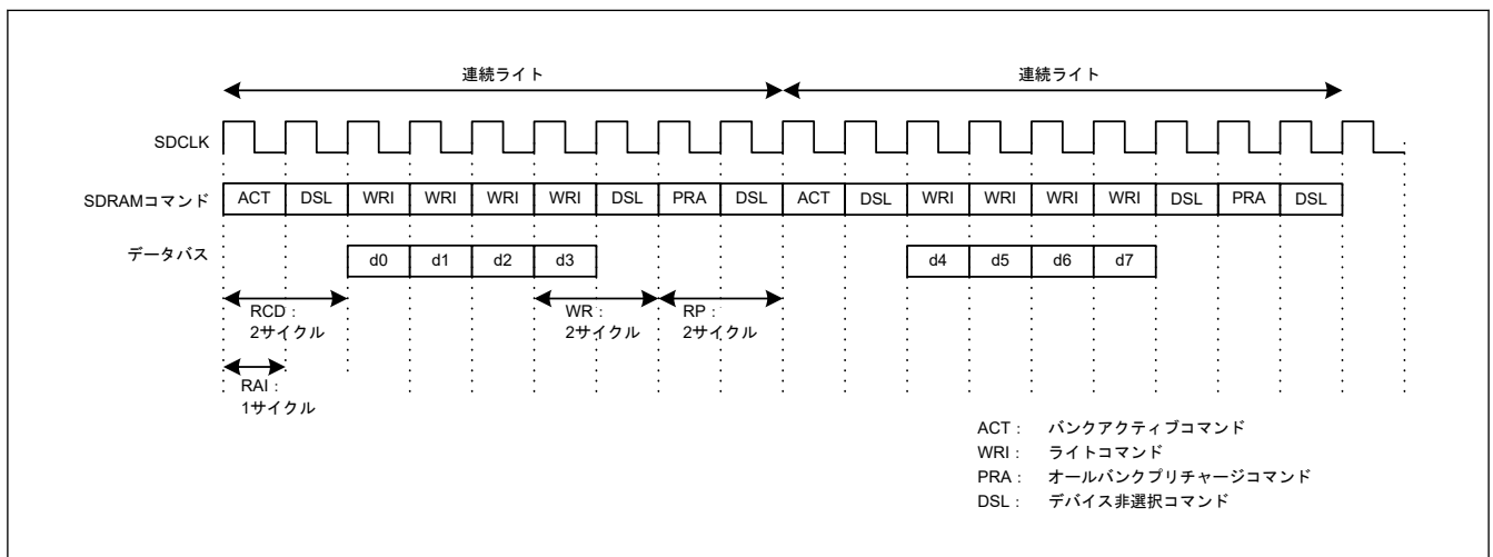
図 14.67 連続ライトタイミング例 (3)
