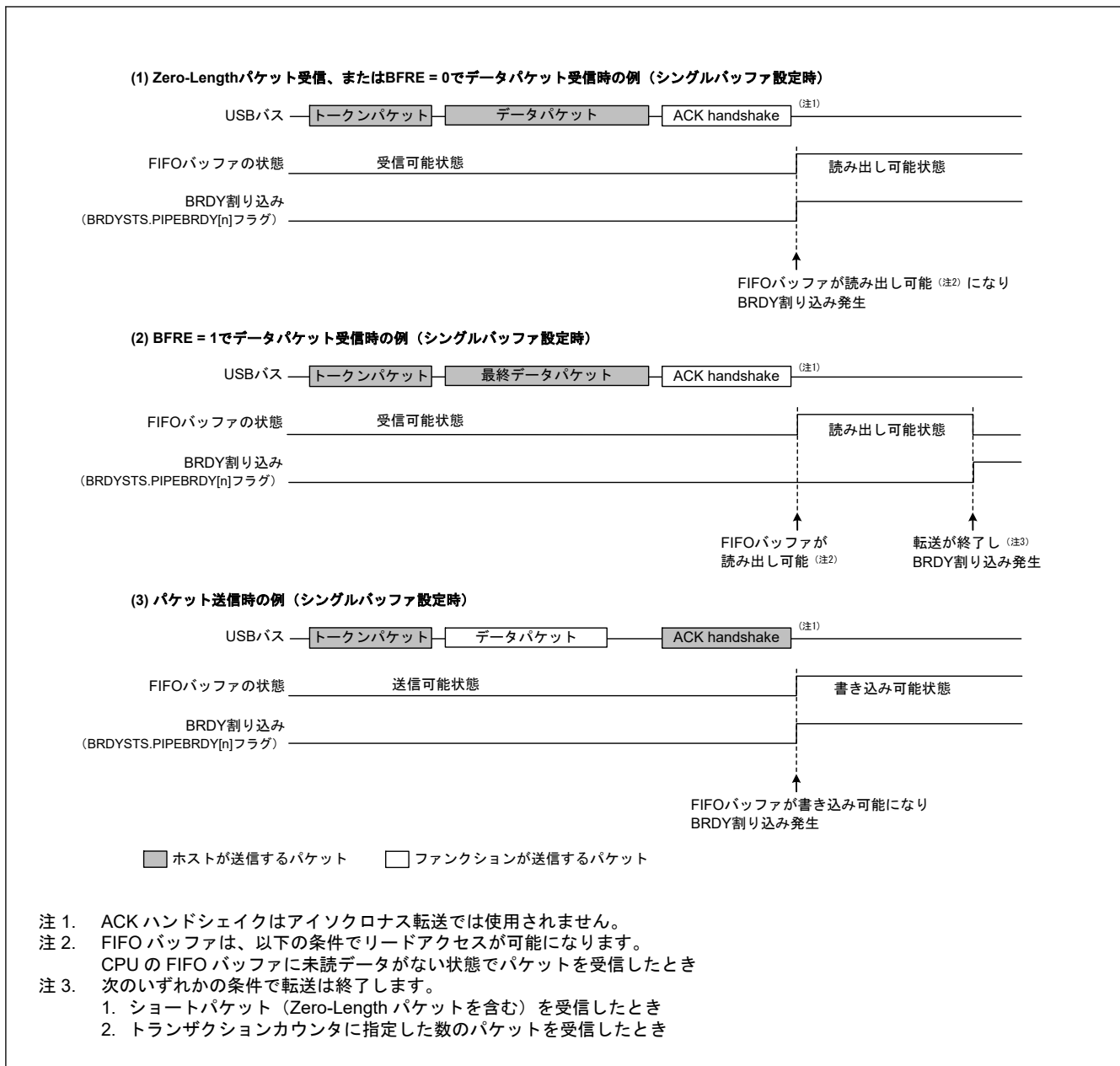
図 30.5 BRDY 割り込み発生タイミング
