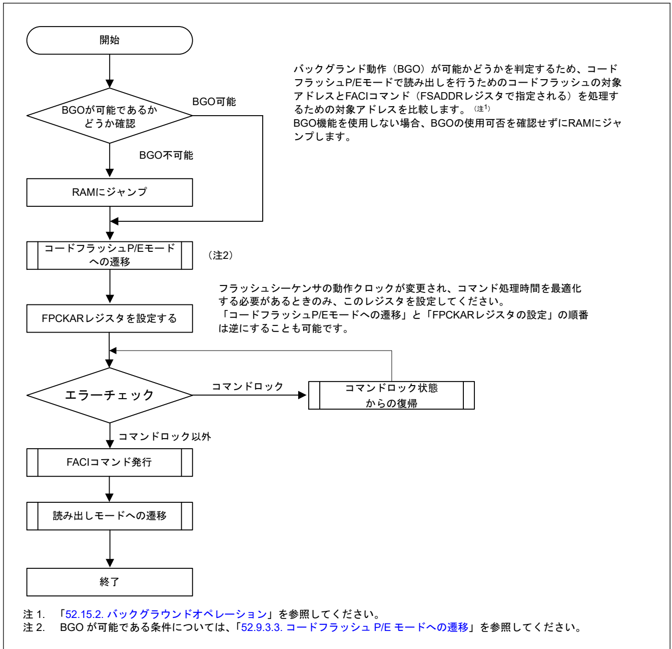
図 52.8 コードフラッシュ P/E モードでのコマンド使用概要
