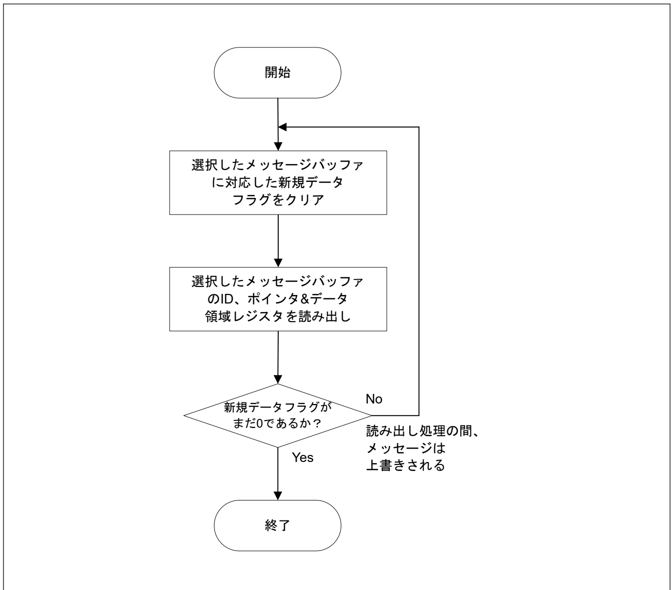
図 34.37 RX メッセージバッファの読み出し手順
