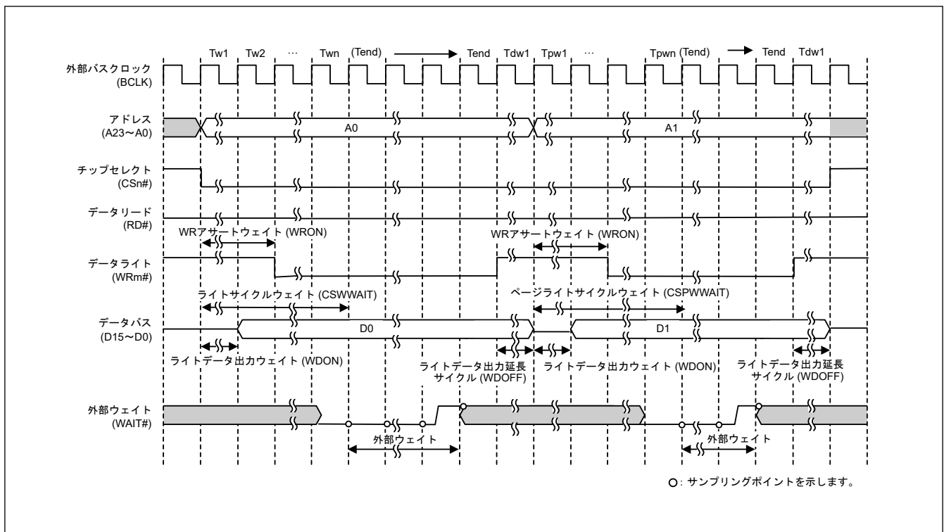
図 14.26 外部ウェイトタイミング例 (バイトストローブモード時の 16 ビットバス空間に対するページライトアクセス、BCLK 端子出力選択ビットで BCLK の 1 分周を選択した場合) (n = 0~7, m = 0, 1)
