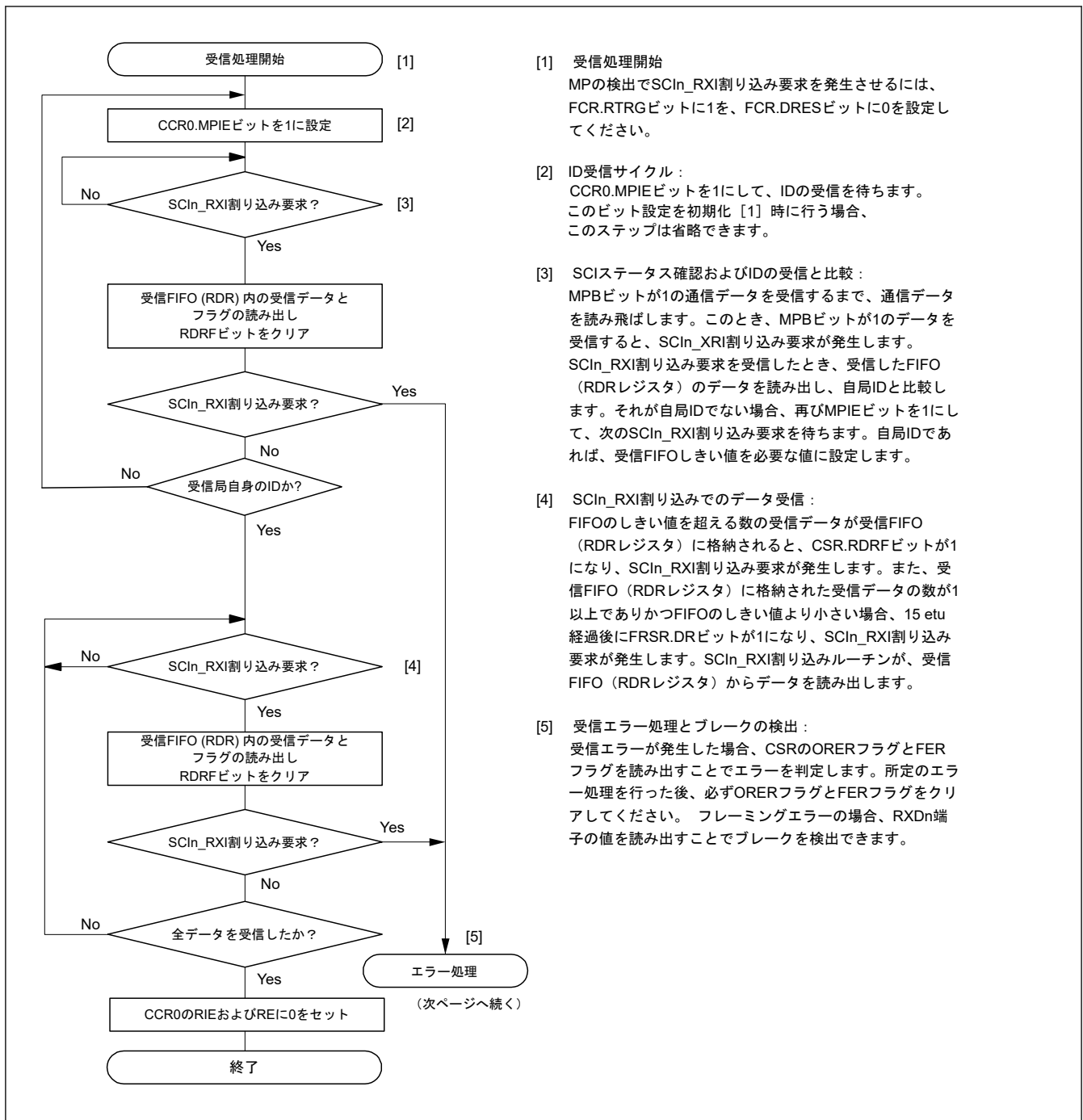
図 31.43 マルチプロセッサモードにおけるシリアル受信のフローチャート例（FIFO 選択時）
