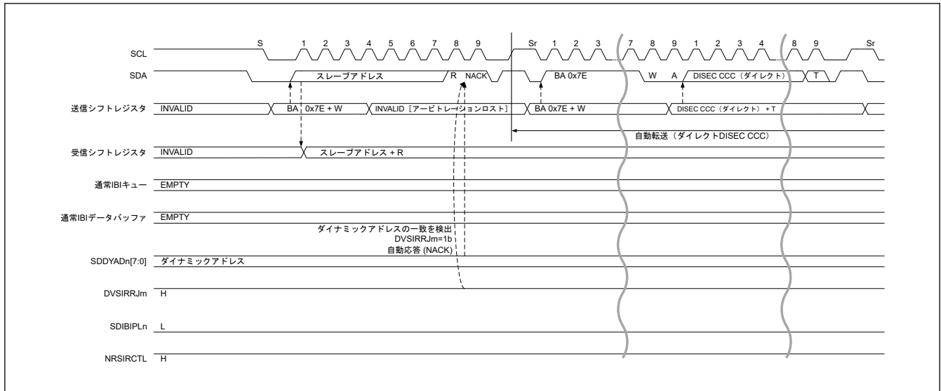
図 33.103 スレーブ割り込み要求 : NACK (DVSIRRJ が 1) かつ NRSIRCTL が 1 の場合 (1/2)
