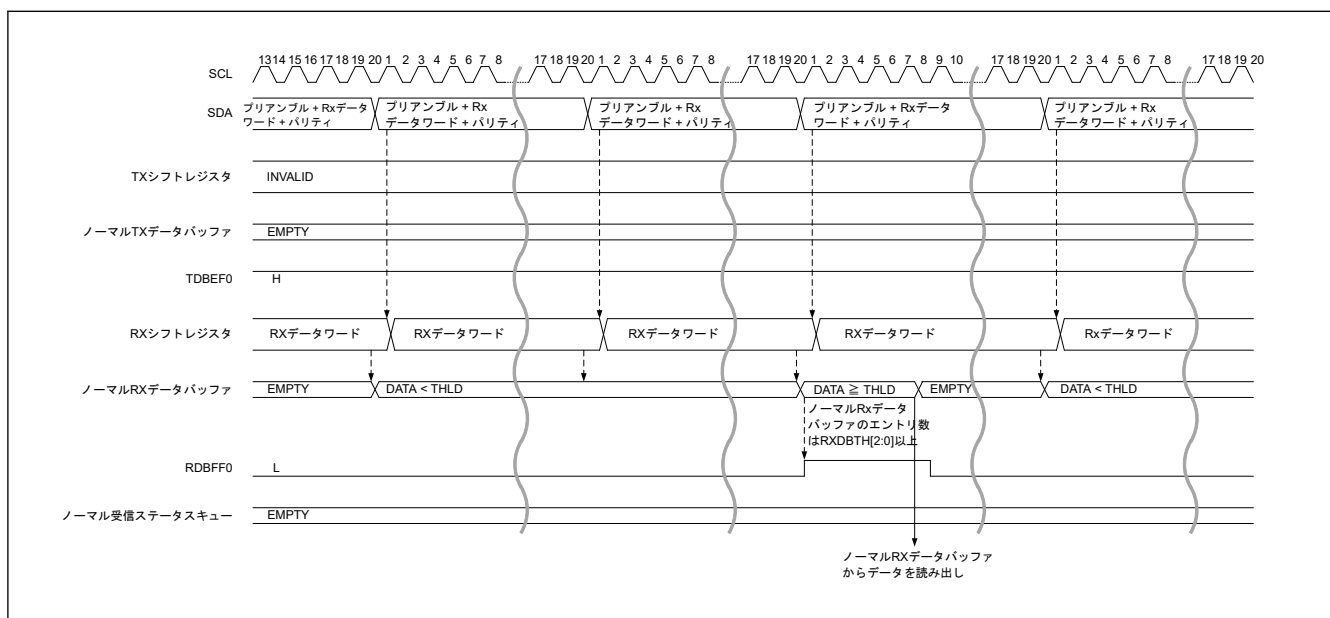
図 33.54 HDR データ書き込み転送 (HDR-DDR) タイミング (2/3)
