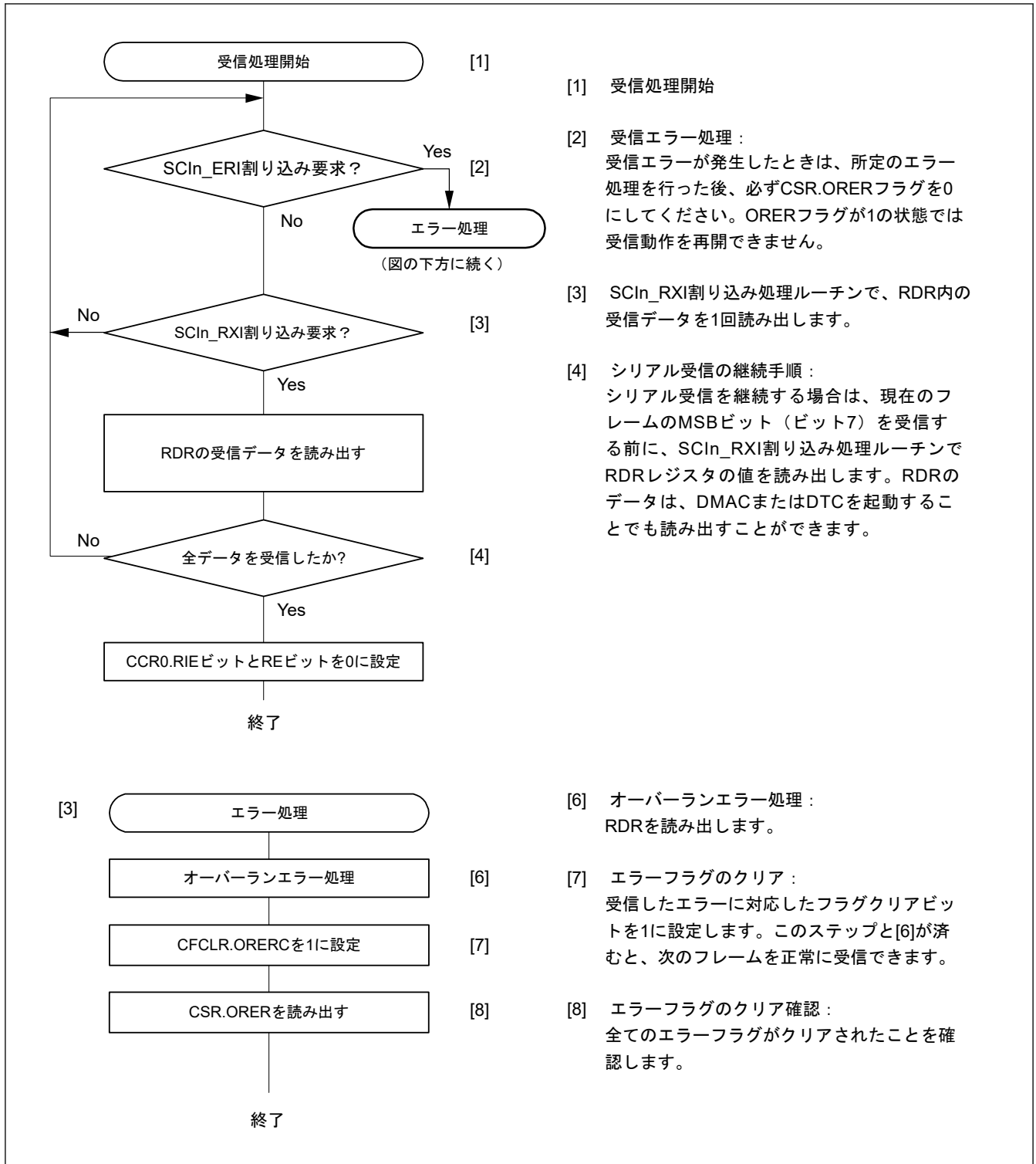
図 31.69 クロック同期式モードにおけるシリアル受信のフローチャート例（非 FIFO 選択時）
