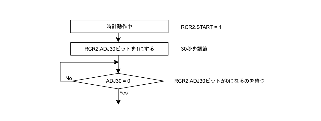
図 24.5 30 秒調整の実行
