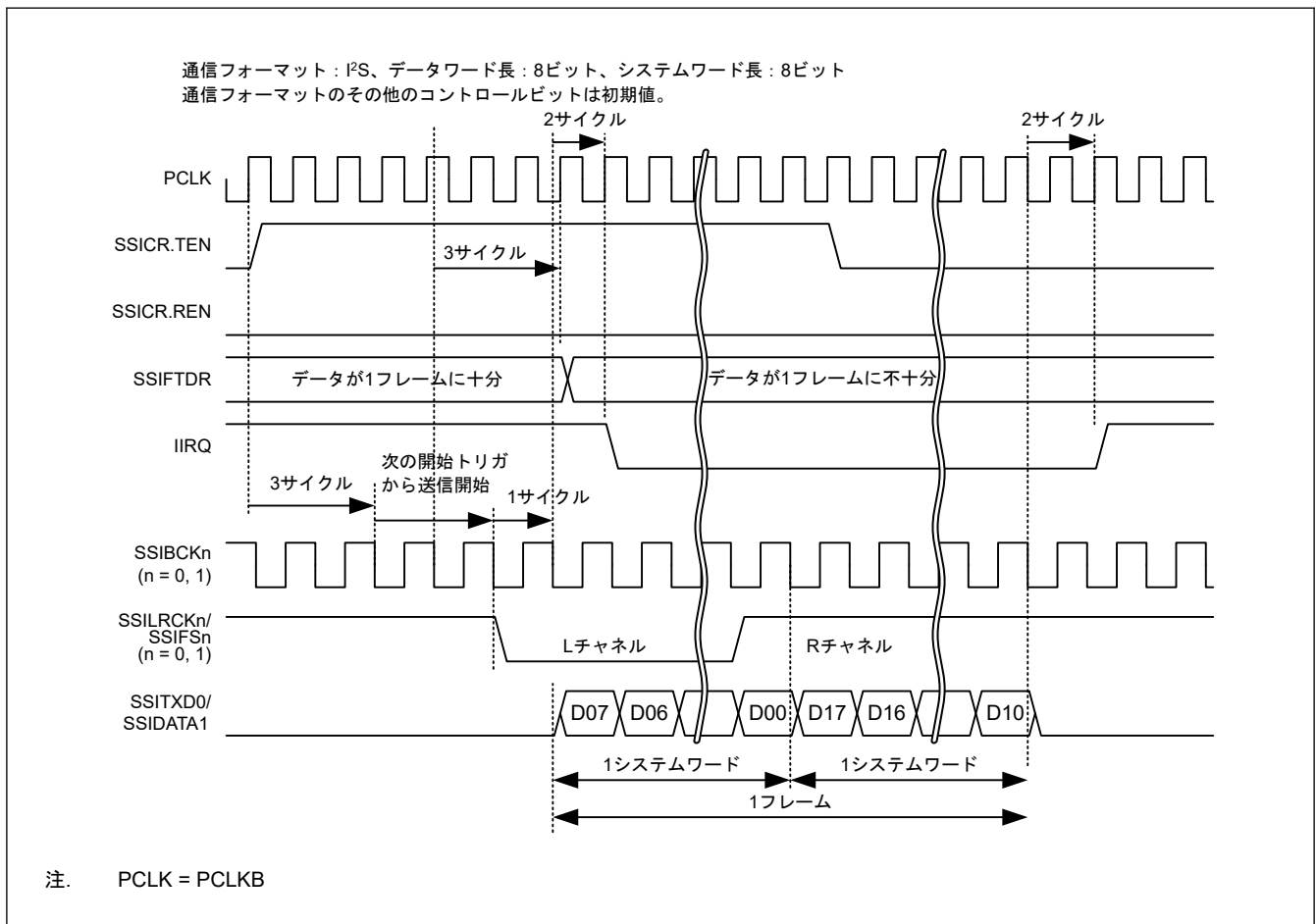
図 39.14 IIRQ 設定タイミング (送信)
