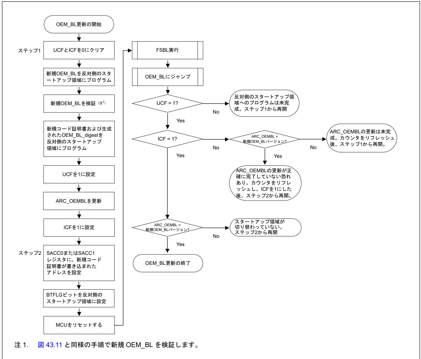
図 43.16 OEM_BL 更新フロー (リニアモード)
