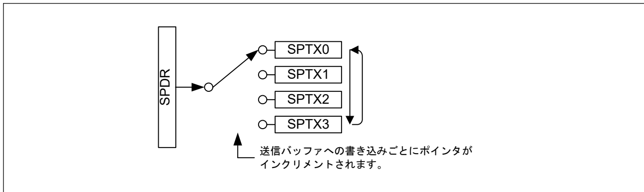
図 36.4 SPDR の構造（書き込み）
