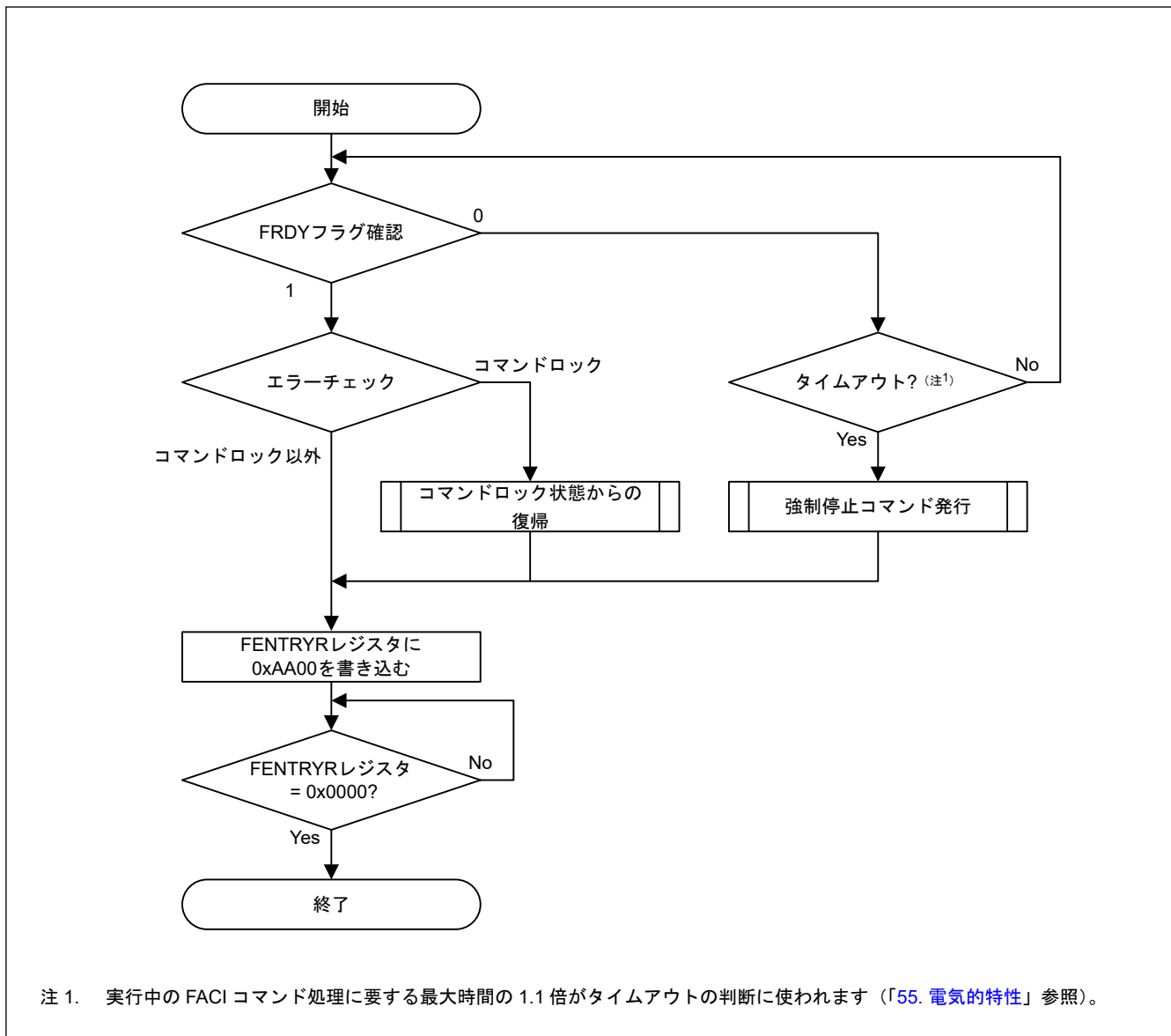
図 52.12 読み出しモードへの遷移手順
