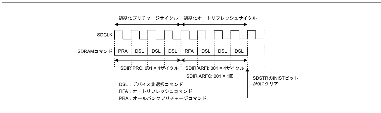
図 14.42 SDRAM 初期化シーケンスのタイミング例
