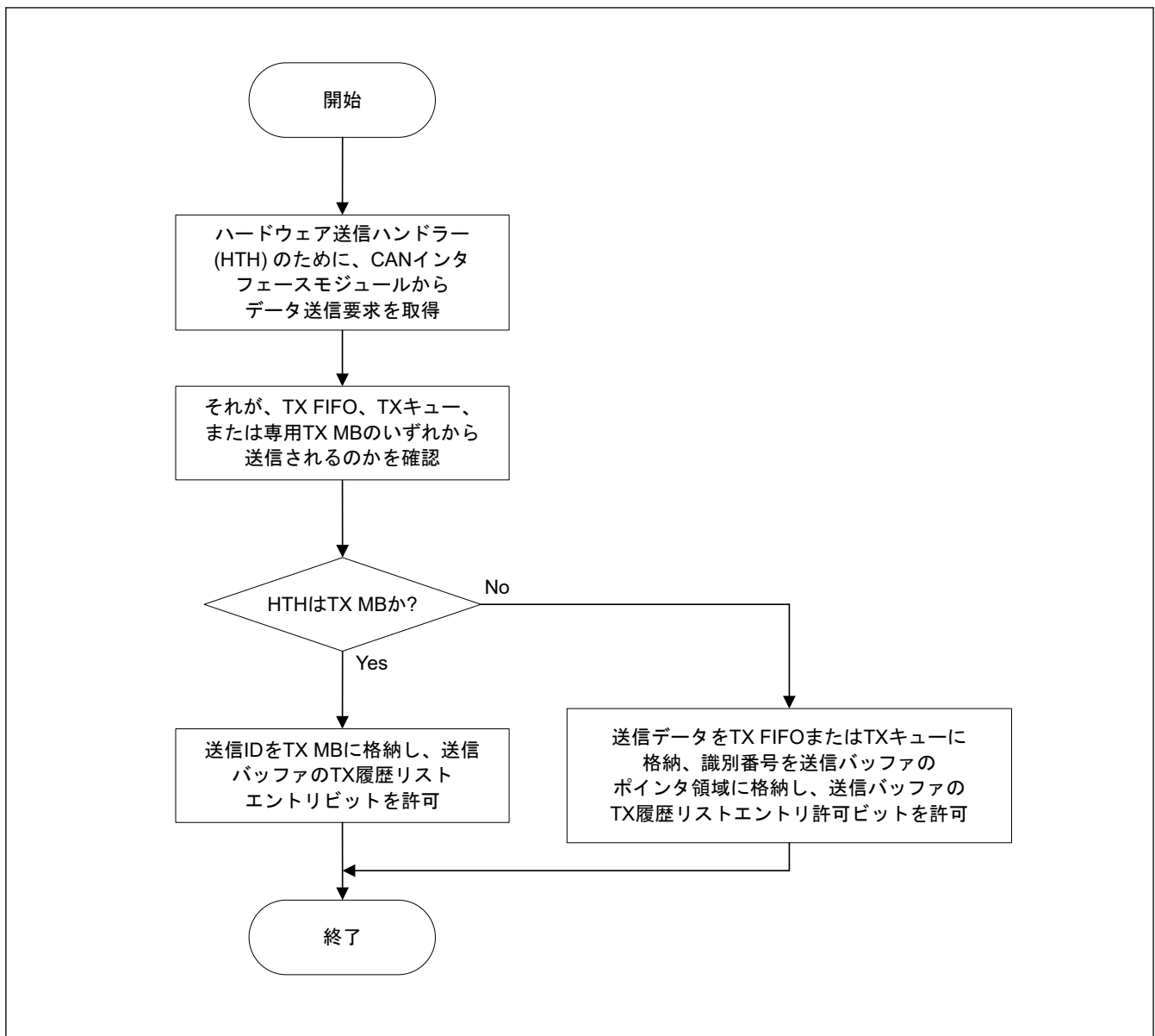
図 34.49 TX履歴リストの準備手順
