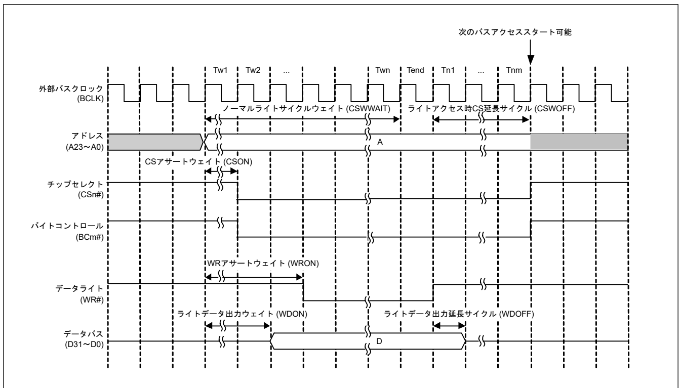
図 14.4 ノーマルライトアクセスのバスタイミング (1 ライトストロブモード) (n = 0~7, m = 0~3)
