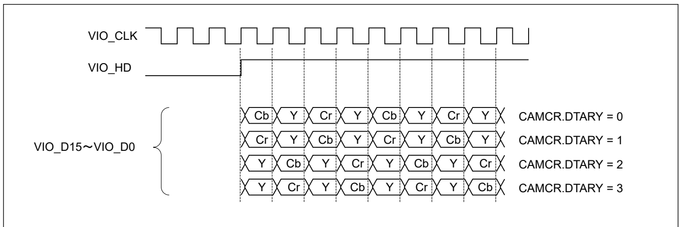
図 53.11 画像データの入力順序
