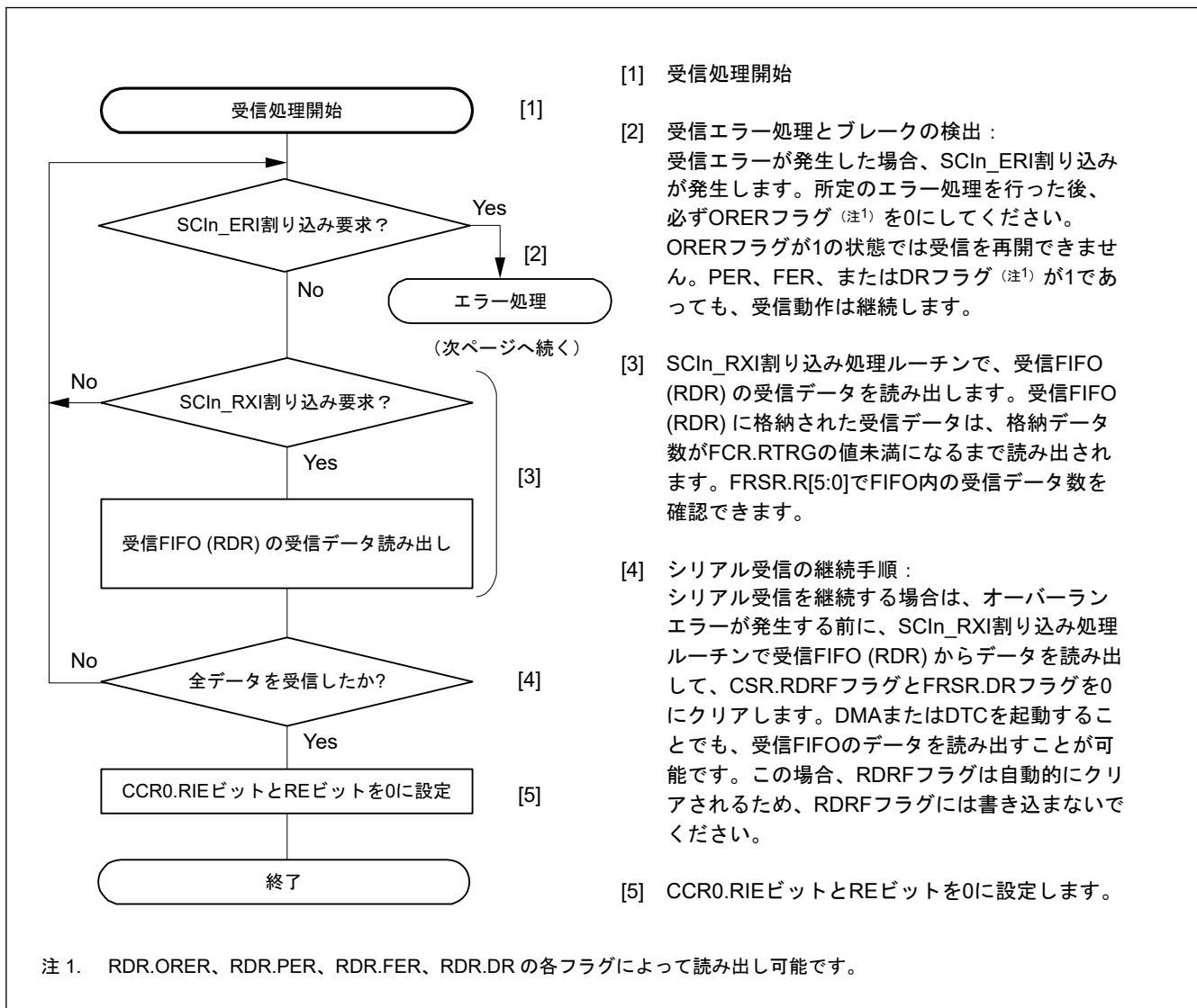
図 31.24 調歩同期式モードにおけるシリアル受信のフローチャート例 (FIFO 選択、アドレス一致検出有効時) (1)
