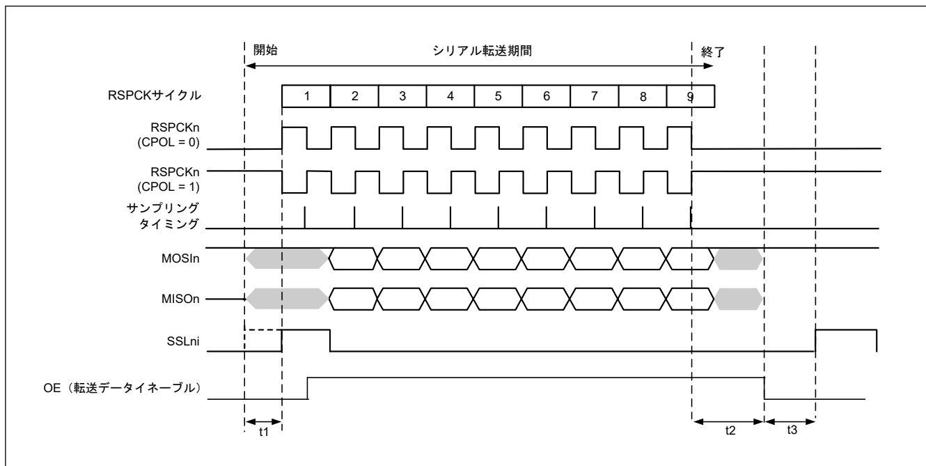
図 36.29 SPI 転送フォーマット (CPHA = 1、SPFRF = 1 の場合)
