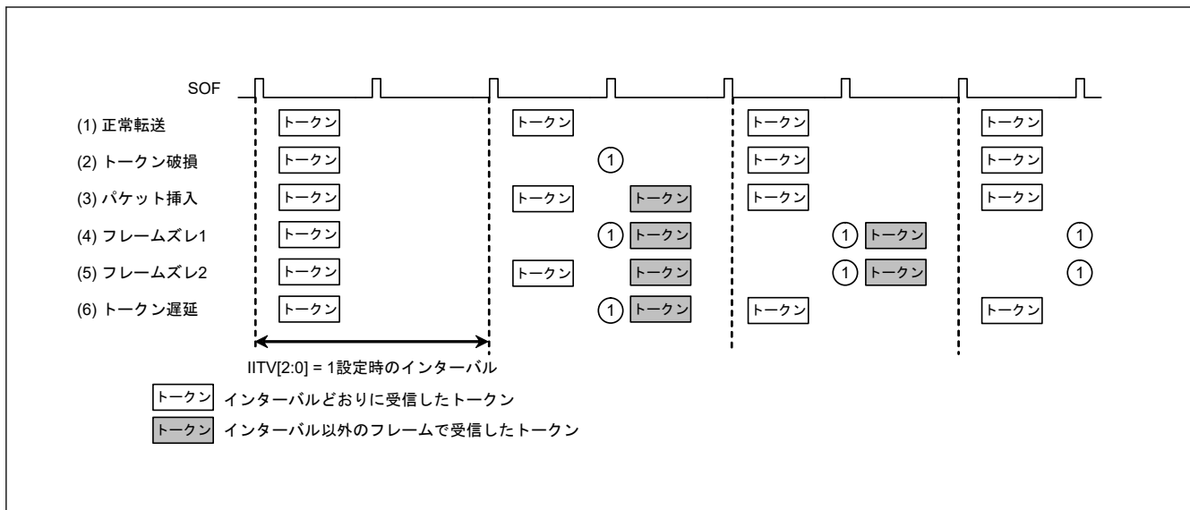
図 30.18 PIPEPERI.IITV[2:0] = 1 の場合のインターバルエラー発生例
