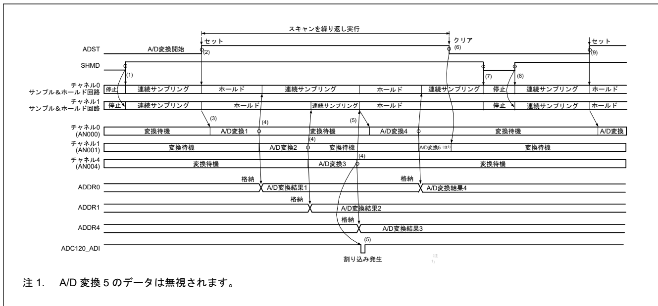
図 45.19 連続スキャンモードの動作例 (チャンネル専用サンプル&ホールド回路使用、AN000、AN001、および AN004 選択、連続サンプリング有効)
