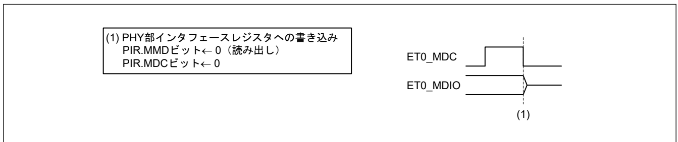
図 27.16 バス解放フロー (表 27.3 の読み出し動作時の TA)
