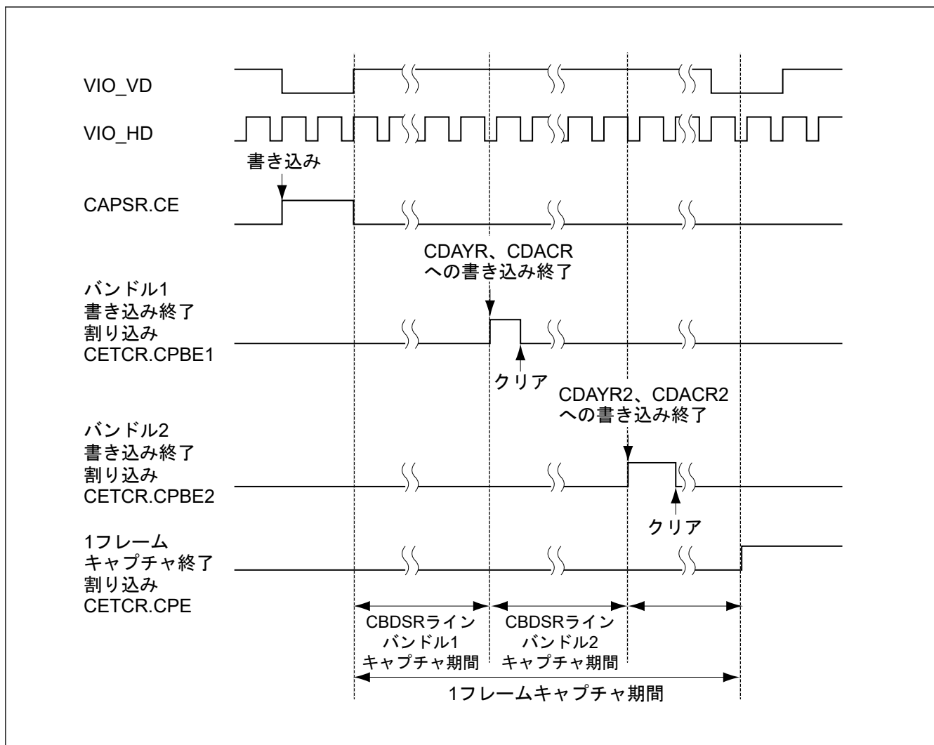
図 53.42 書き込み終了割り込みのタイミング (画像キャプチャ時、データ同期取り込み時)
