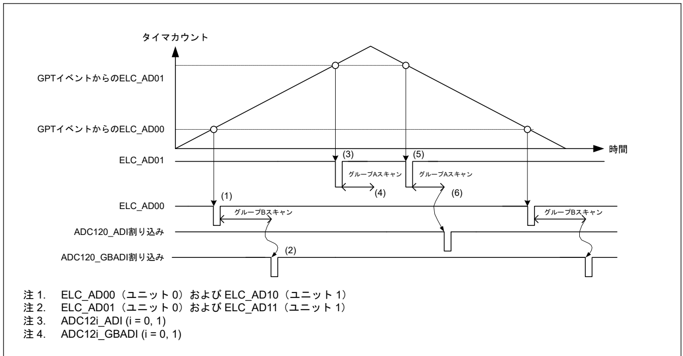
図 45.25 グループスキャンモードでダブルトリガモードを使用する場合の基本動作例 (ELC からの同期トリガ使用時)
