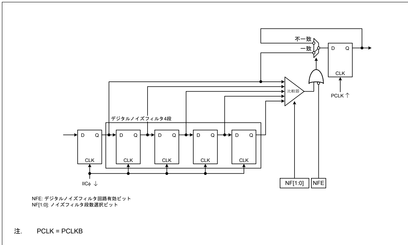
図 32.23 デジタルノイズフィルタ回路のブロック図
