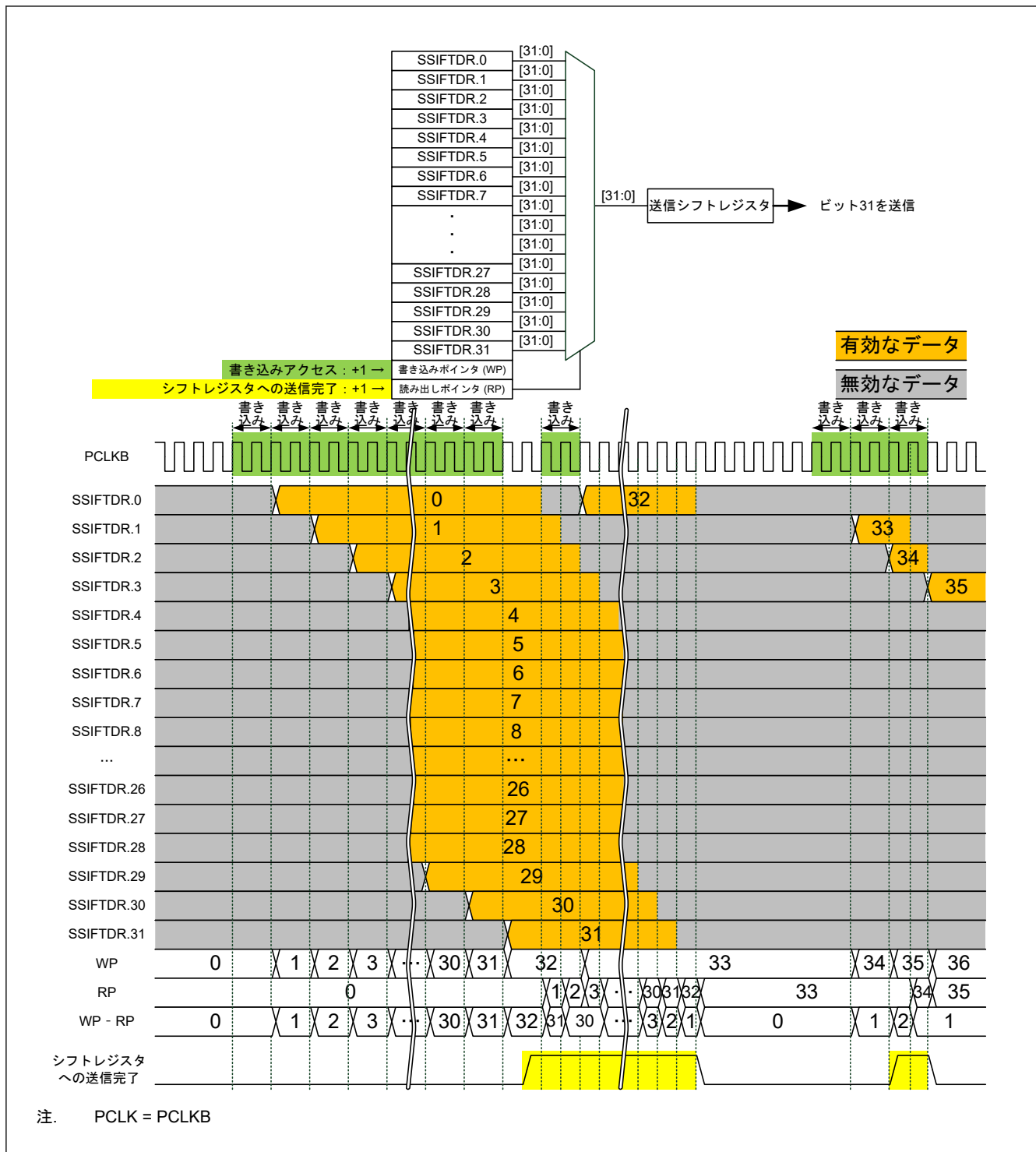
図 39.31 送信 FIFO データレジスタと送信シフトレジスタの構成、および FIFO の動作例
