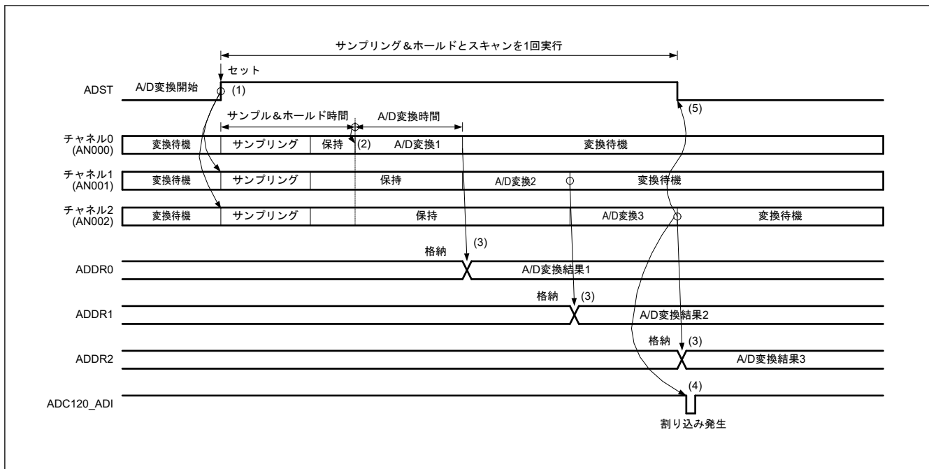
図 45.9 シングルスキャンモードの動作例 (チャンネル専用サンプル&ホールド回路使用、AN000~AN002 選択)
