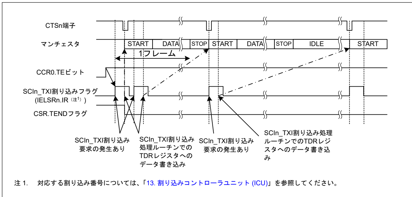
図 31.53 マンチェスタモードにおけるシリアル送信の送信開始動作の例 (プレフィスなし、CTS 機能あり)
