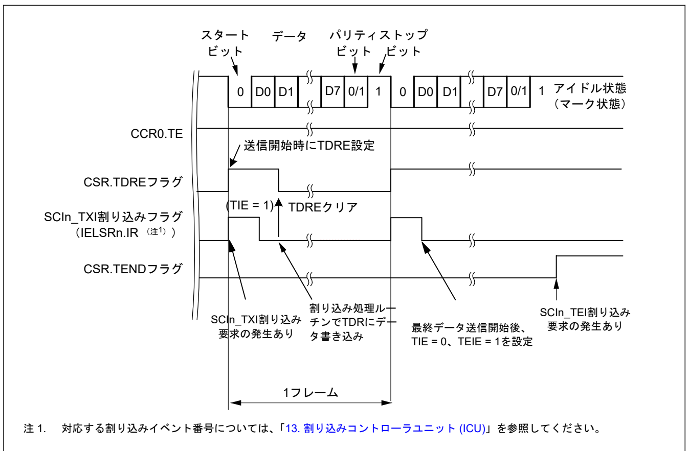
図 31.14 調歩同期式モードにおけるシリアル送信の動作例 (3) (8 ビットデータ/パリティあり/1ストップビット/CTS 機能不使用/送信途中~送信完了時)
