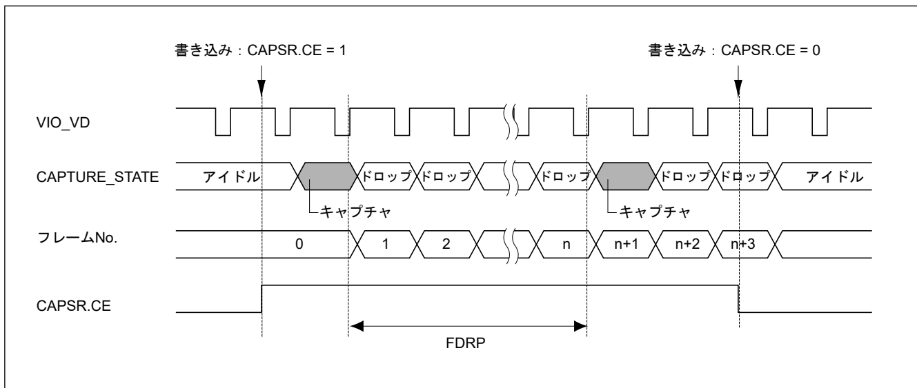
図 53.9 FDRP ビットの設定値とフレームドロップタイミング
