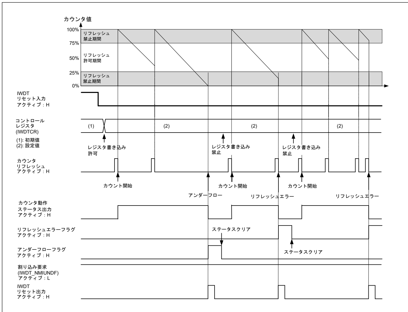
図 26.3 レジスタスタートモードでの動作例
