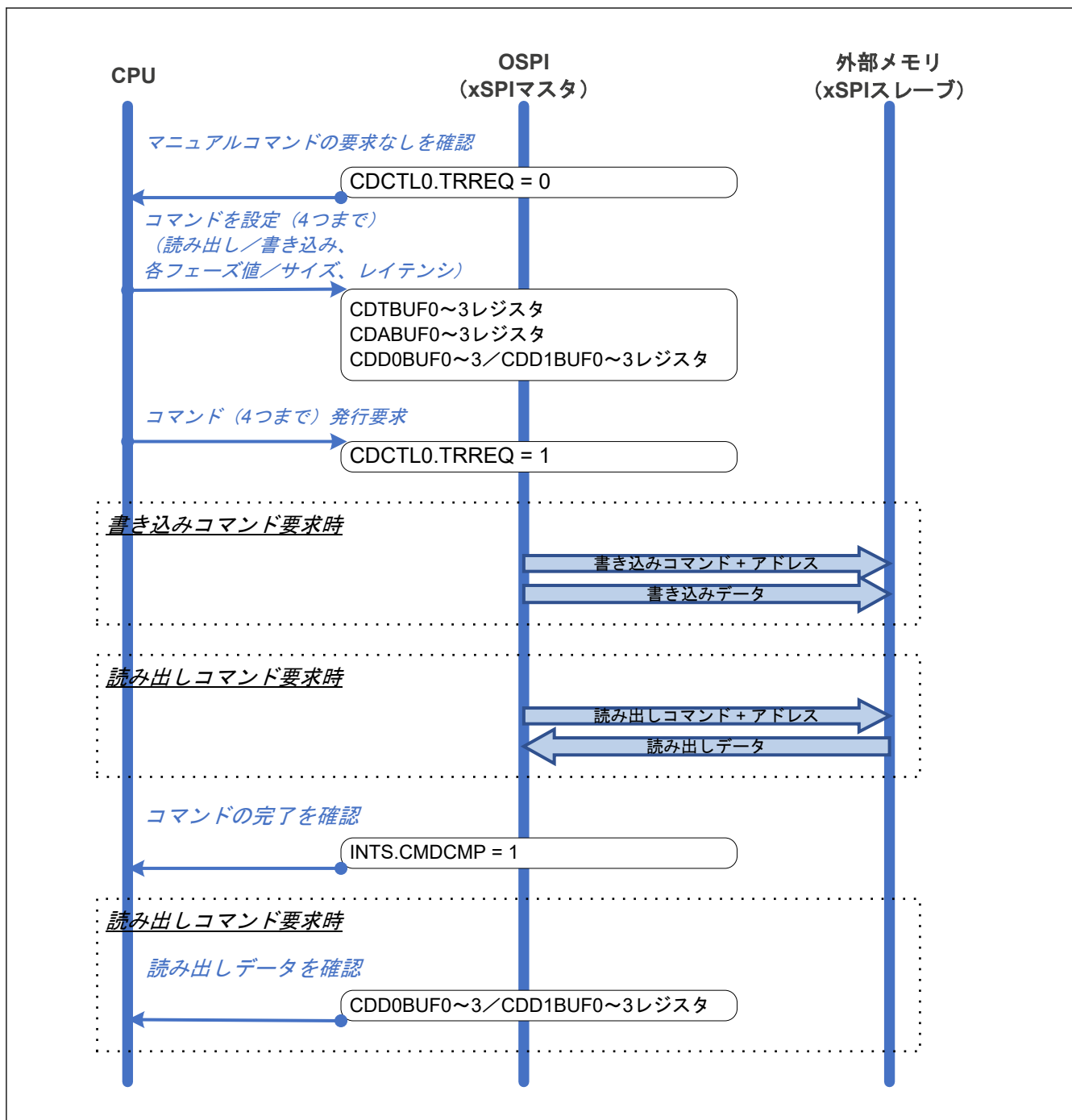
図 37.25 マニュアルコマンド手順のフロー (直接モード)
