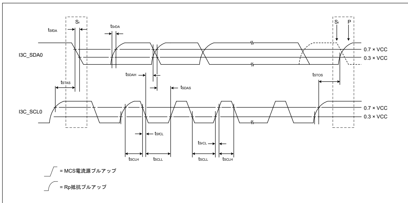
図 55.73 I 2 C バスインタフェース入出力タイミング (Hs モード)
