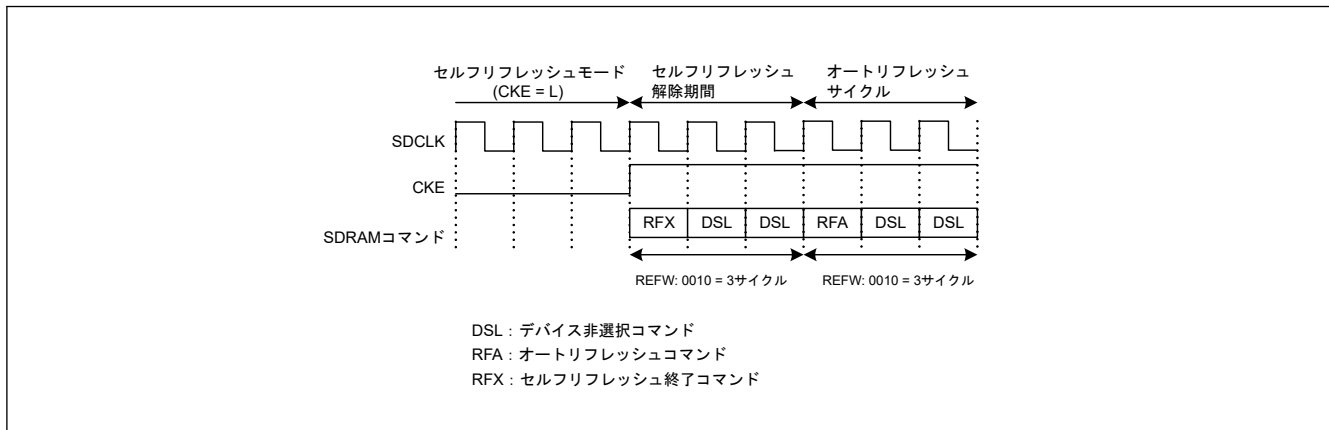
図 14.38 セルフリフレッシュモードからの復帰タイミング例
