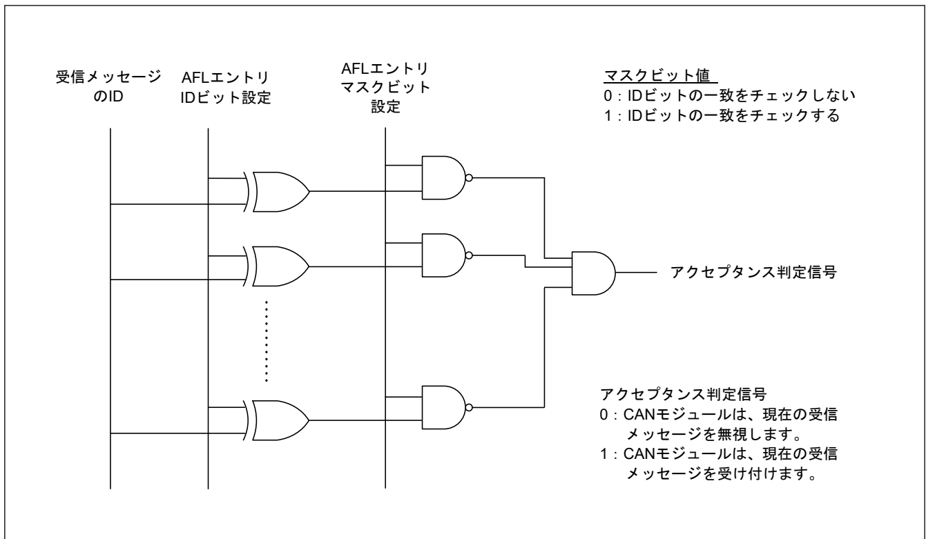
図 34.25 アクセプタンス機能
