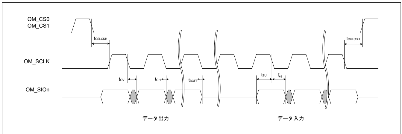
図 55.67 SDR 送受信タイミング (1S-1S-1S、1S-2S-2S、2S-2S-2S、1S-4S-4S、4S-4S-4S)
