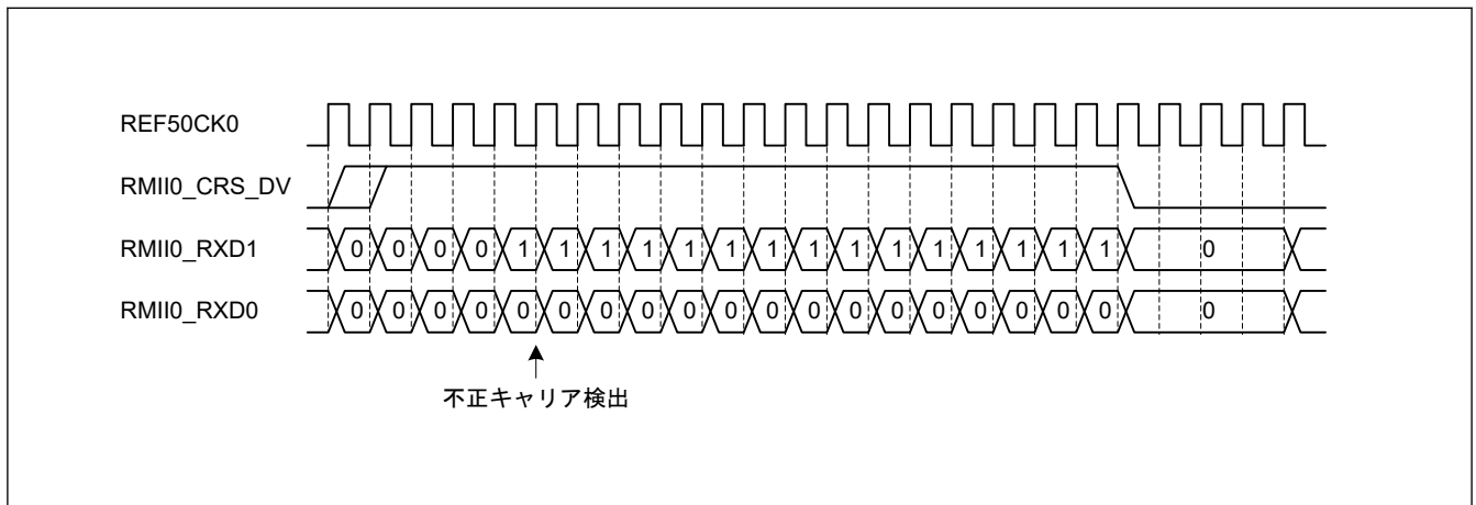
図 27.14 RMII フレーム受信タイミング (不正キャリア検出時)
