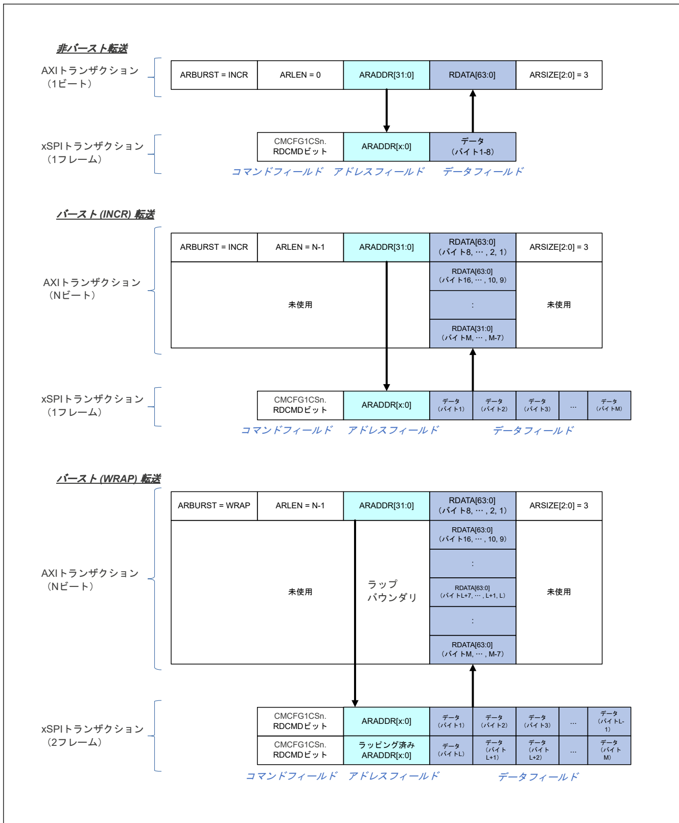
図 37.17 読み出しアクセス時の xSPI フレームのフォーマット (通常フォーマット)
