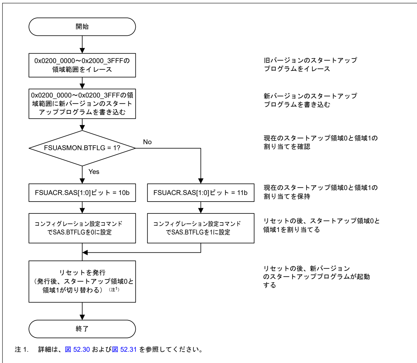
図 52.32 スタートアッププログラムプロテクションの概念 (セキュアエアリアスの場合)
