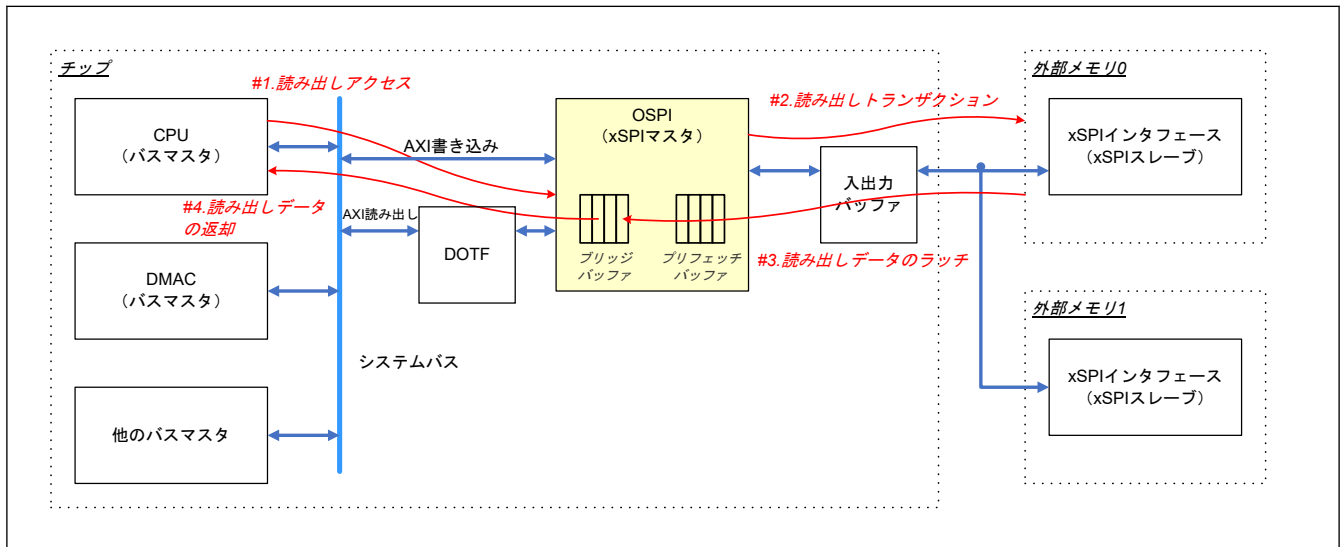
図 37.16 メモリ領域に対する読み出しアクセス
