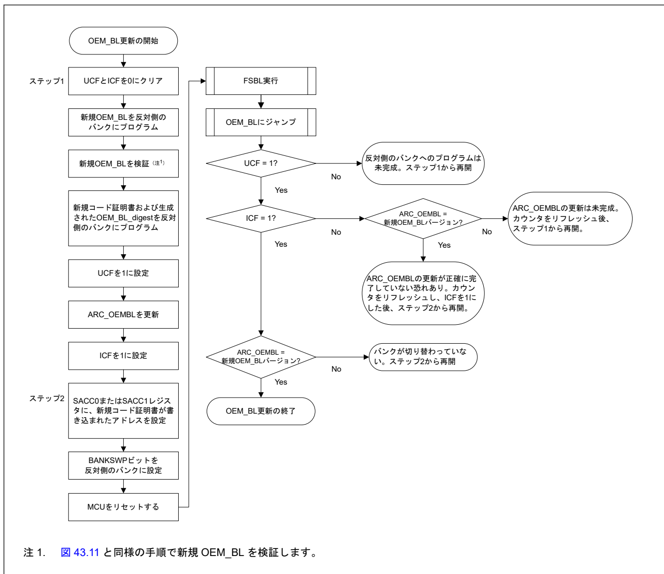
図 43.15 OEM_BL 更新フロー (デュアルモード)
