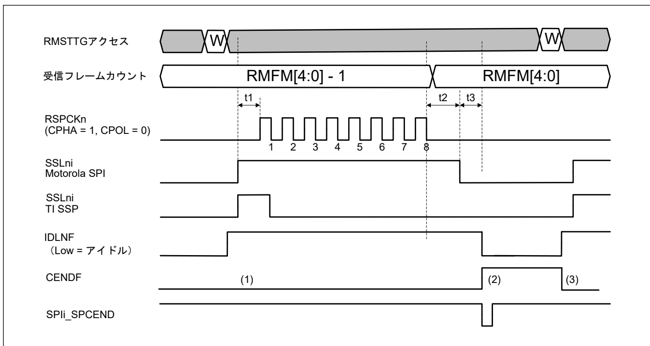
図 36.39 RMFM[4:0] ≠ 0 時の通信終了割り込み動作例 (受信専用マスタモード/Motorola-SPI)
