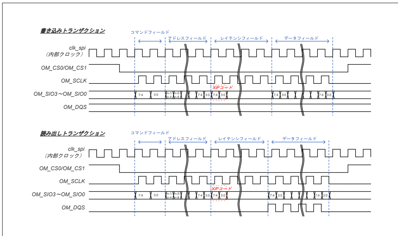
図 37.5 4S-4D-4D のタイミングチャート
