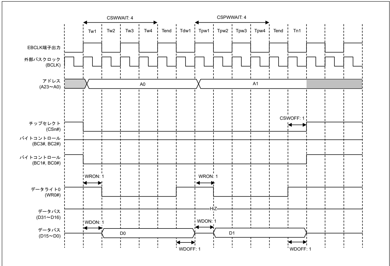
図 14.20 ページライトアクセスの動作例 (EBCLK 端子出力選択ビットで BCLK の 2 分周を設定した場合、および 1 転送要求に対して 2 回バスアクセスが発生する場合、1 ライトストローブモード時) (n = 0~7)
