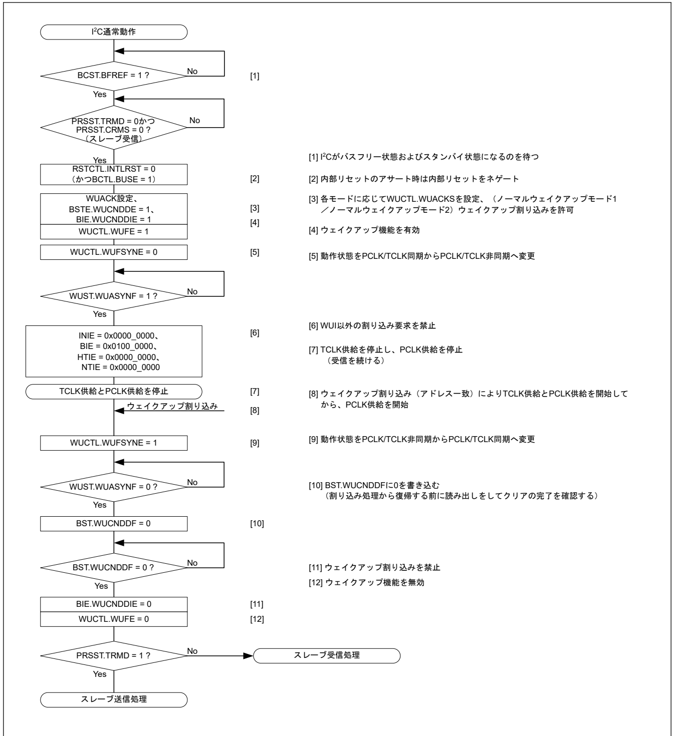
図 33.129 ノーマル WU モード 2 の使用例 (スレーブアドレス一致に起因するウェイクアップ割り込みによるウェイクアップリカバリの場合)
