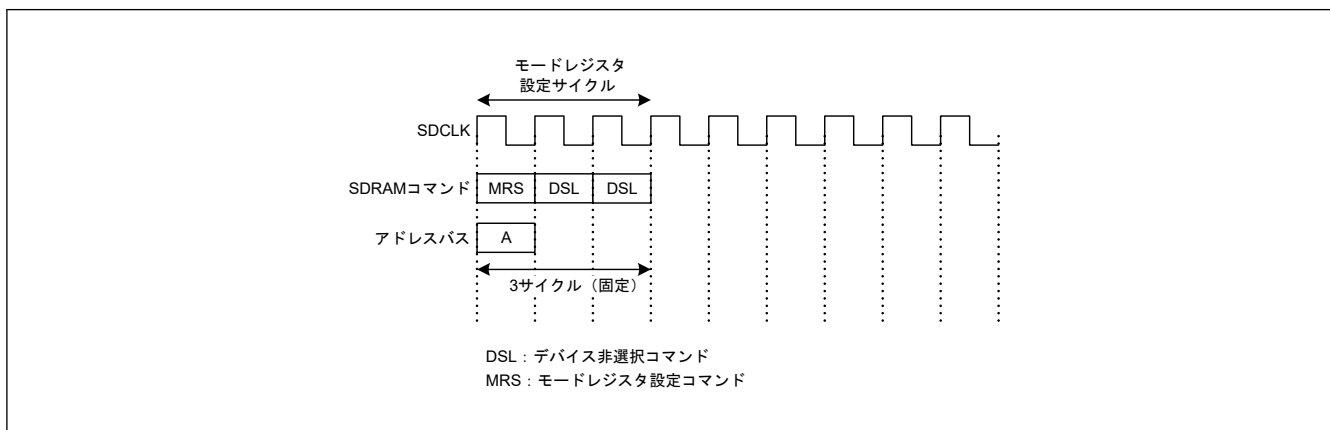
図 14.48 モードレジスタ設定動作タイミング
