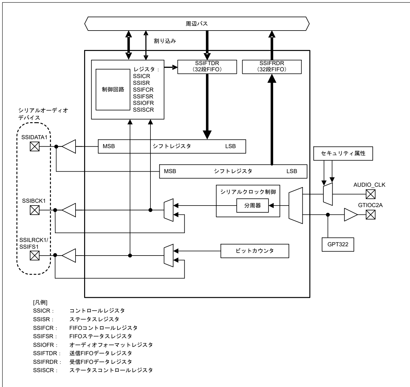
図 39.3 SSIE ブロック図 (SSIE1)
