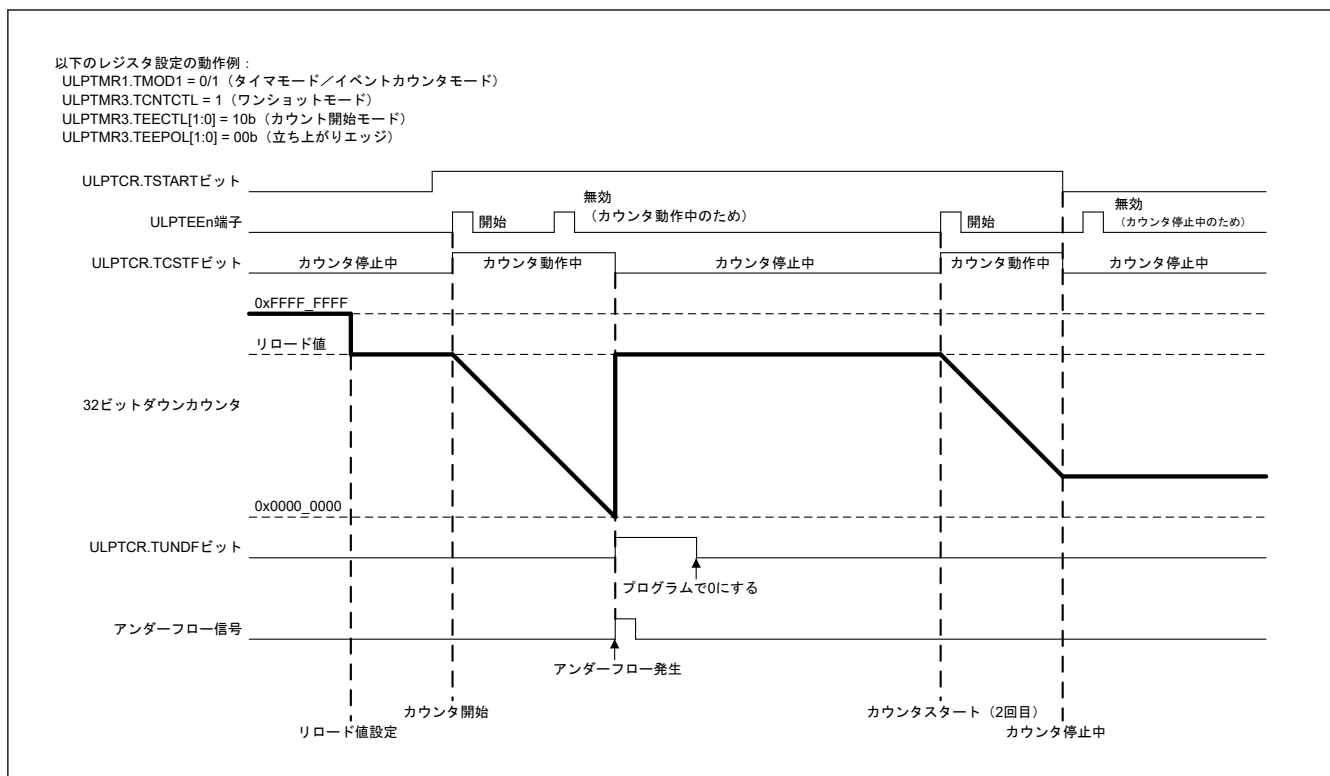
図 23.11 共通&ワンショット&カウント開始モードでの動作例
