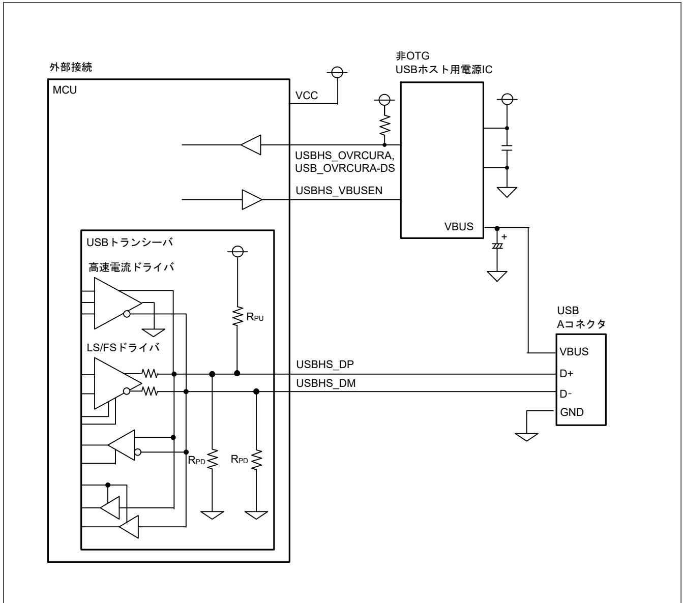
図 30.30 USB ホスト接続例
