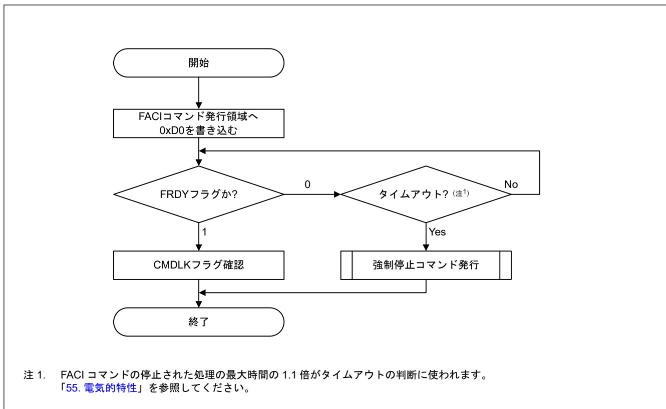
図 52.21 P/E レジュームコマンドの使用フロー
