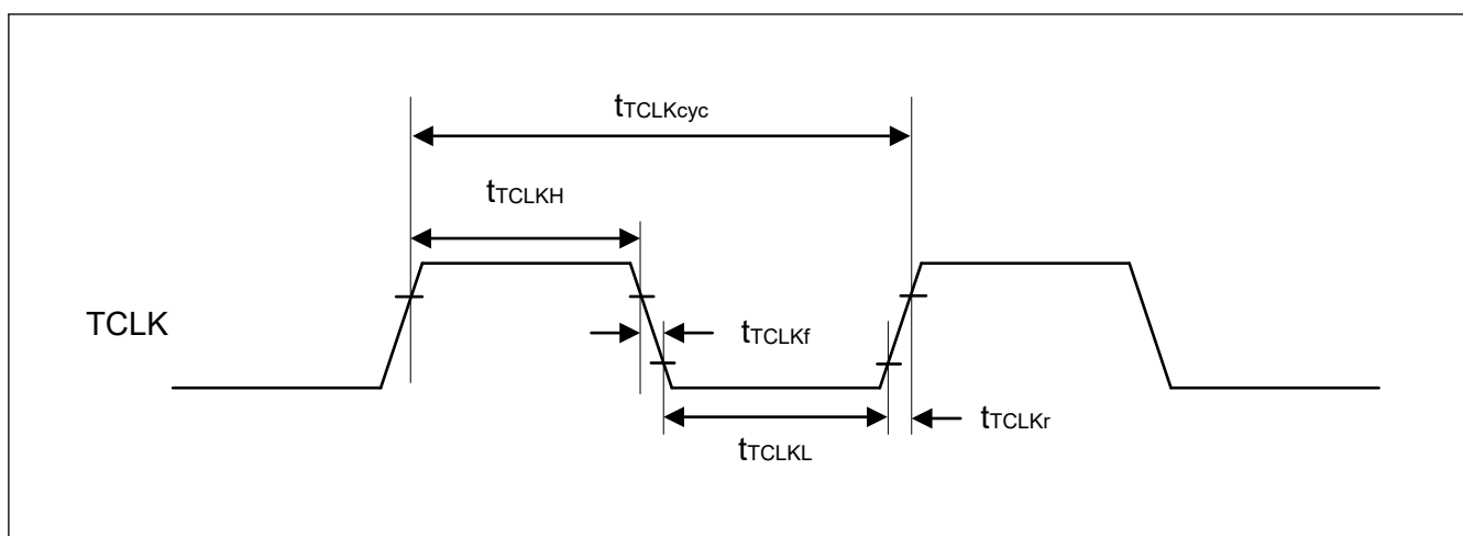
図 55.132 ETM TCLK タイミング
