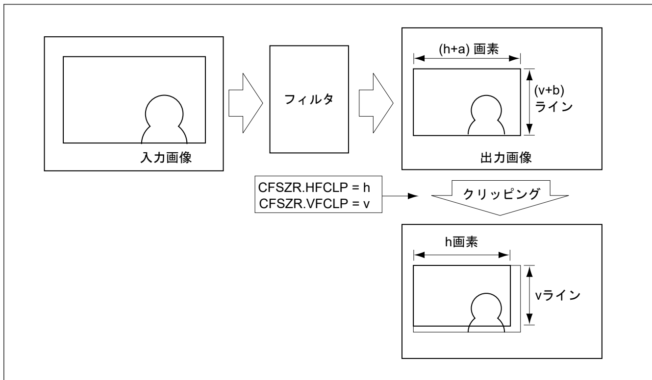
図 53.33 フィルタ出力画像のクリッピング
