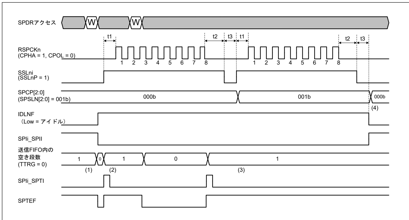
図 36.34 アイドル割り込み動作の例 (マスターモード/Motorola-SPI)
