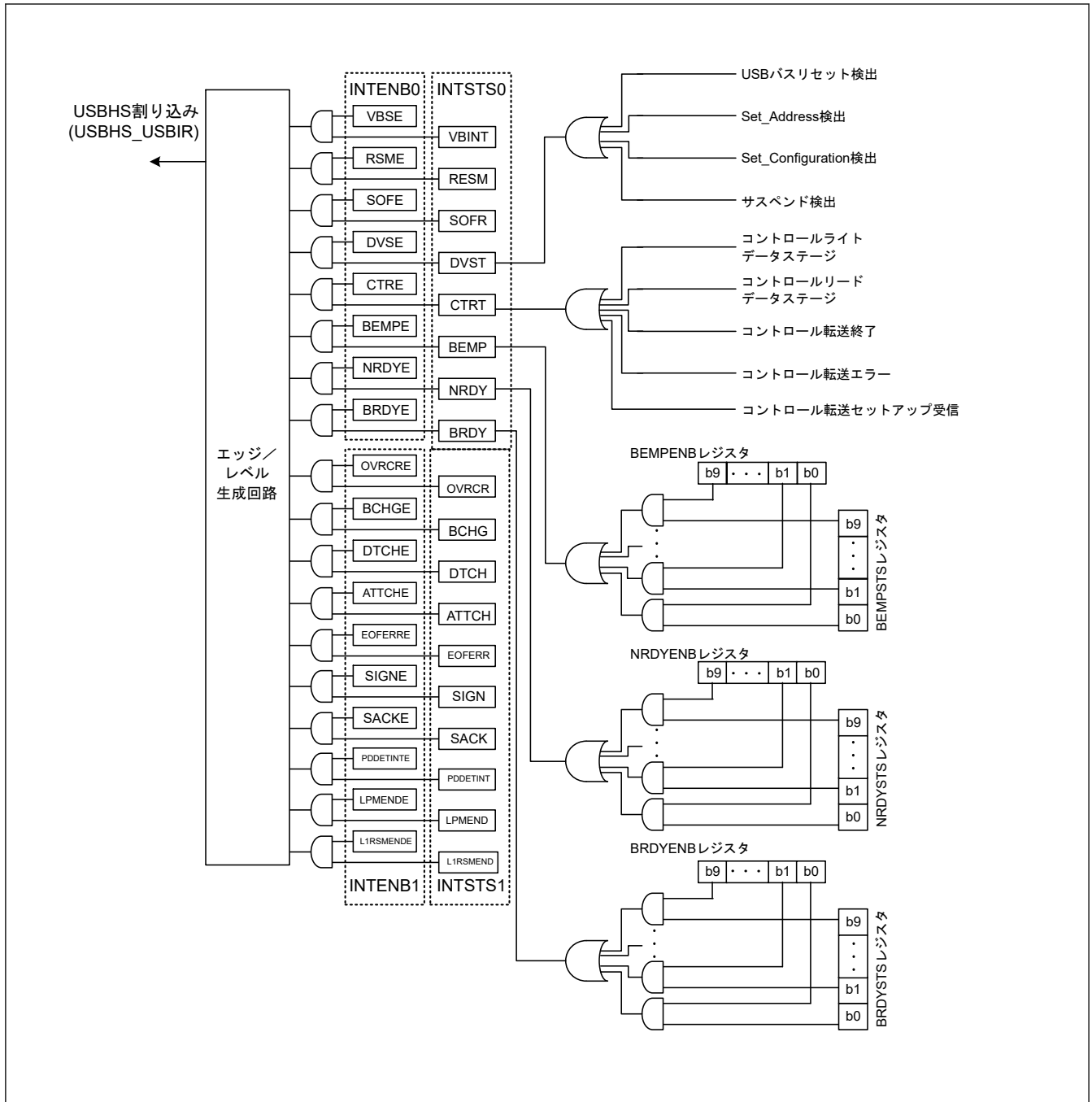
図 30.4 USBHS 割り込み関連回路
