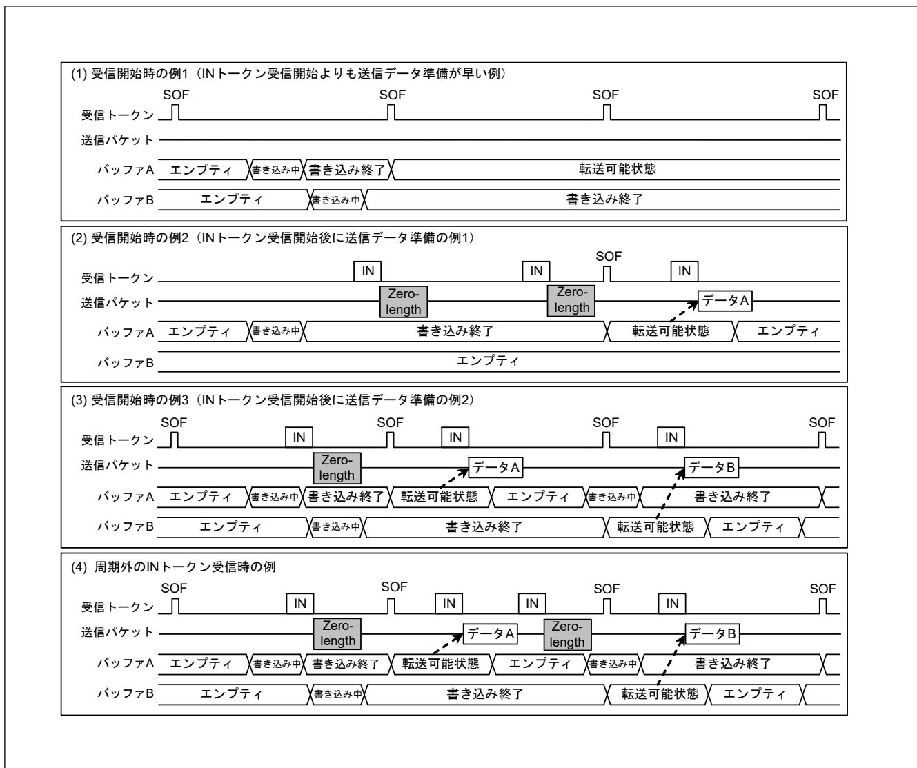
図 30.16 データセットアップ動作例
