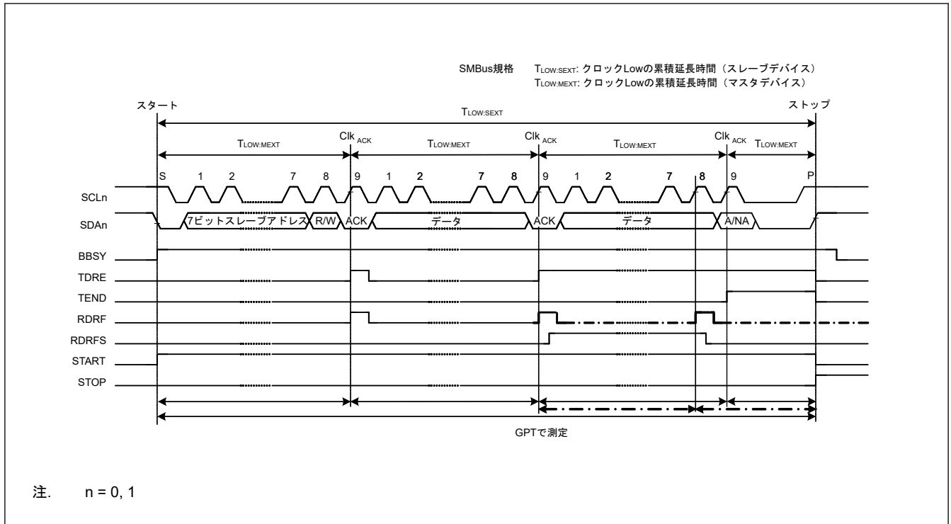
図 32.50 SMBus タイムアウト測定
