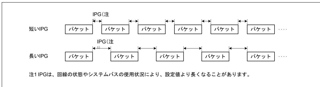
図 27.19 IPG の変化による伝送効率の違い
