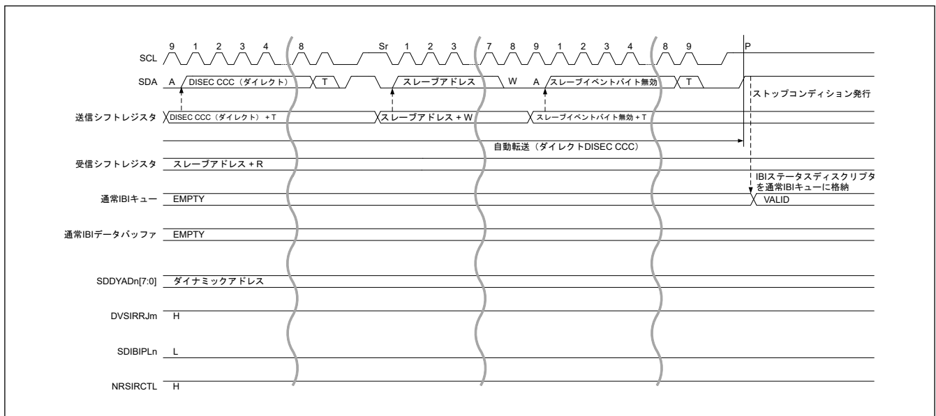
図 33.104 スレーブ割り込み要求 : NACK (DVSIRRJ が 1) かつ NRSIRCTL が 1 の場合 (2/2)
