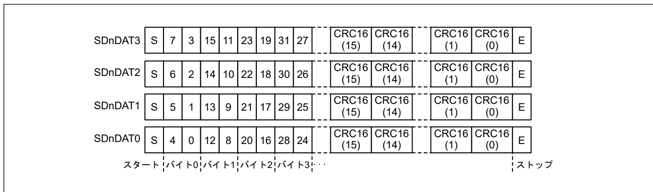
図 40.3 4 ビット幅モードの SDnDAT
