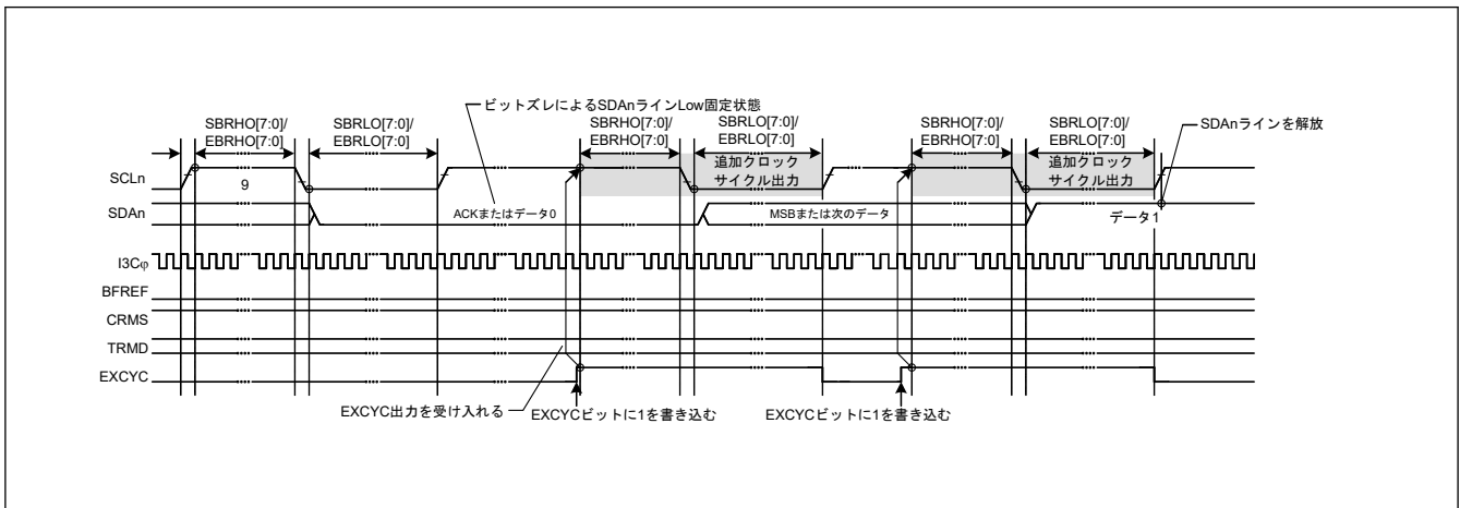
図 33.113 SCL クロック追加出力機能 (EXCYC ビット)
