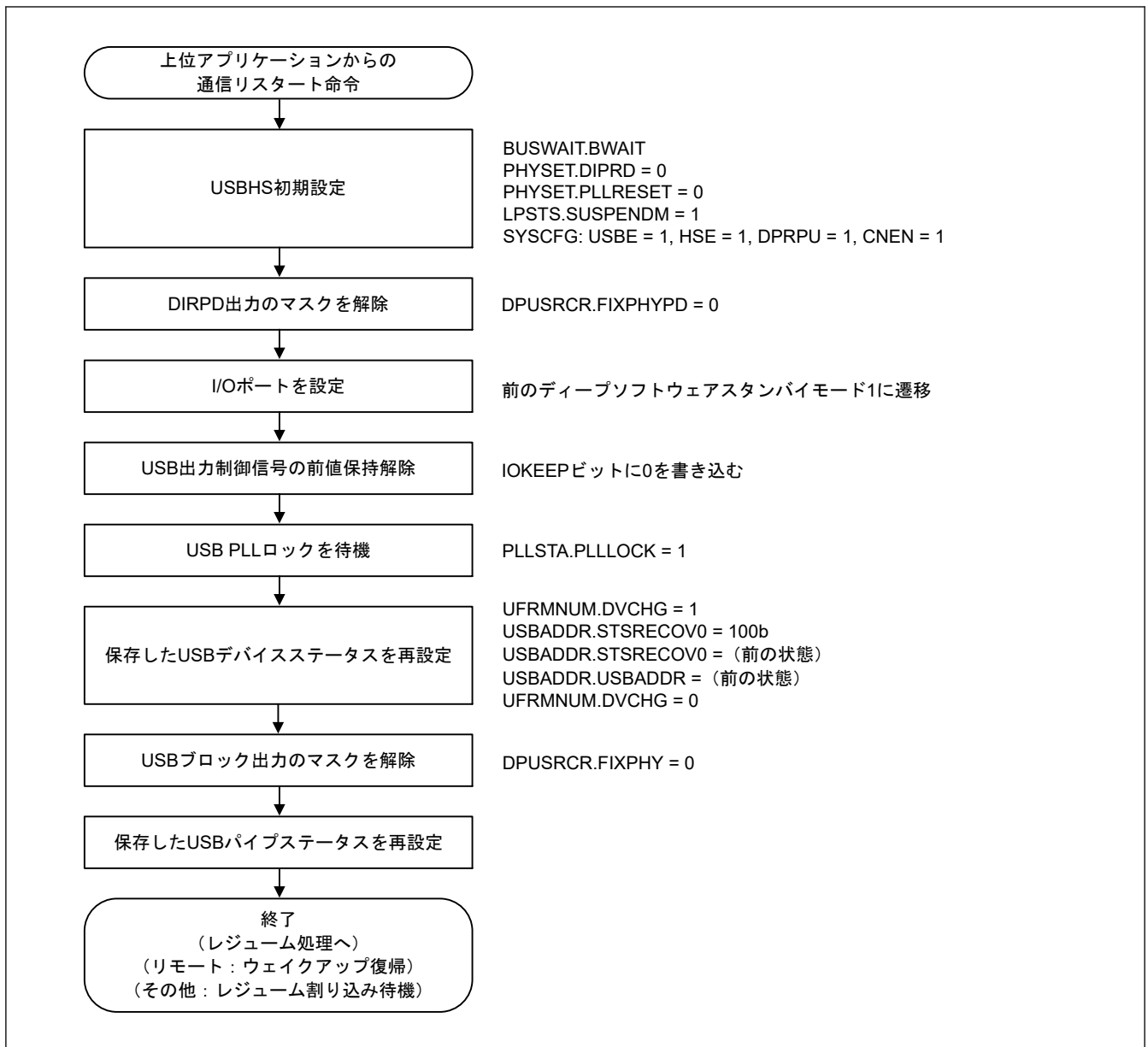
図 30.26 デバイスコントローラとしてディープソフトウェアスタンバイモード1を解除する場合のUSBHS設定フロー (2)
