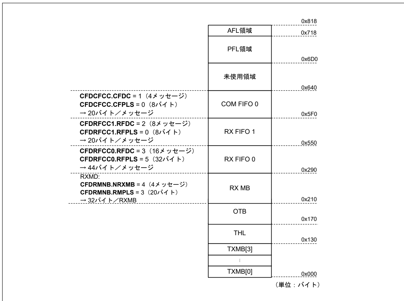
図 34.55 RX MB + FIFO バッファの RAM 領域の構成例
