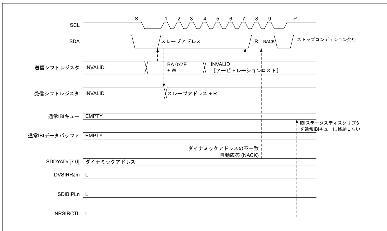
図 33.102 スレーブ割り込み要求 : NACK (DAT.SDDYAD[7:0]ビットが一致しない) かつ NRSIRCTL が 0 の場合
