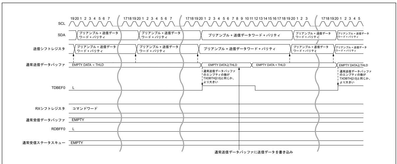
図 33.59 HDR データ読み出し転送 (HDR-DDR) タイミング (2/3)
