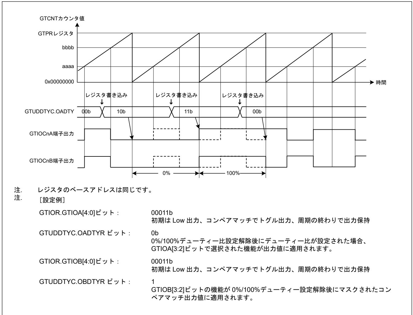
図 21.31 出力デューティー 0%、100%機能動作例
