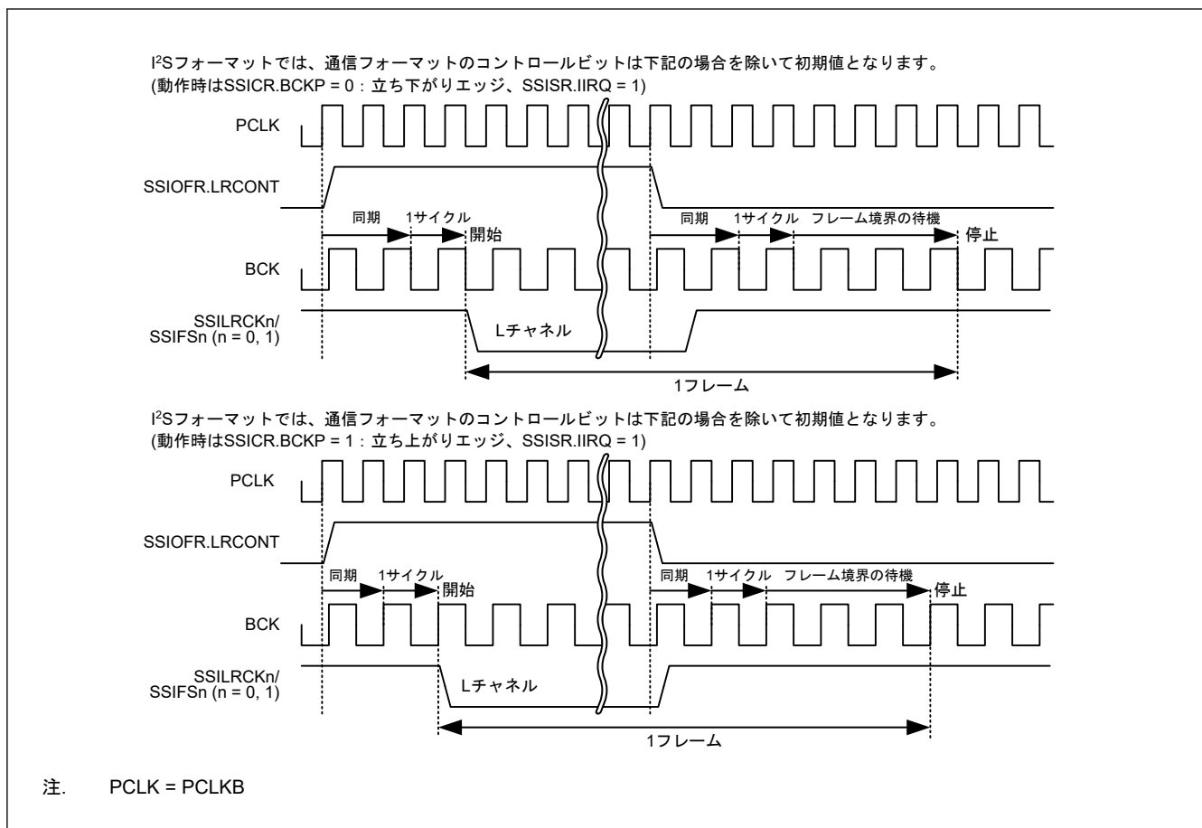
図 39.44 SSI OFR.LRCONT による LR クロック/フレーム同期継続禁止の例
