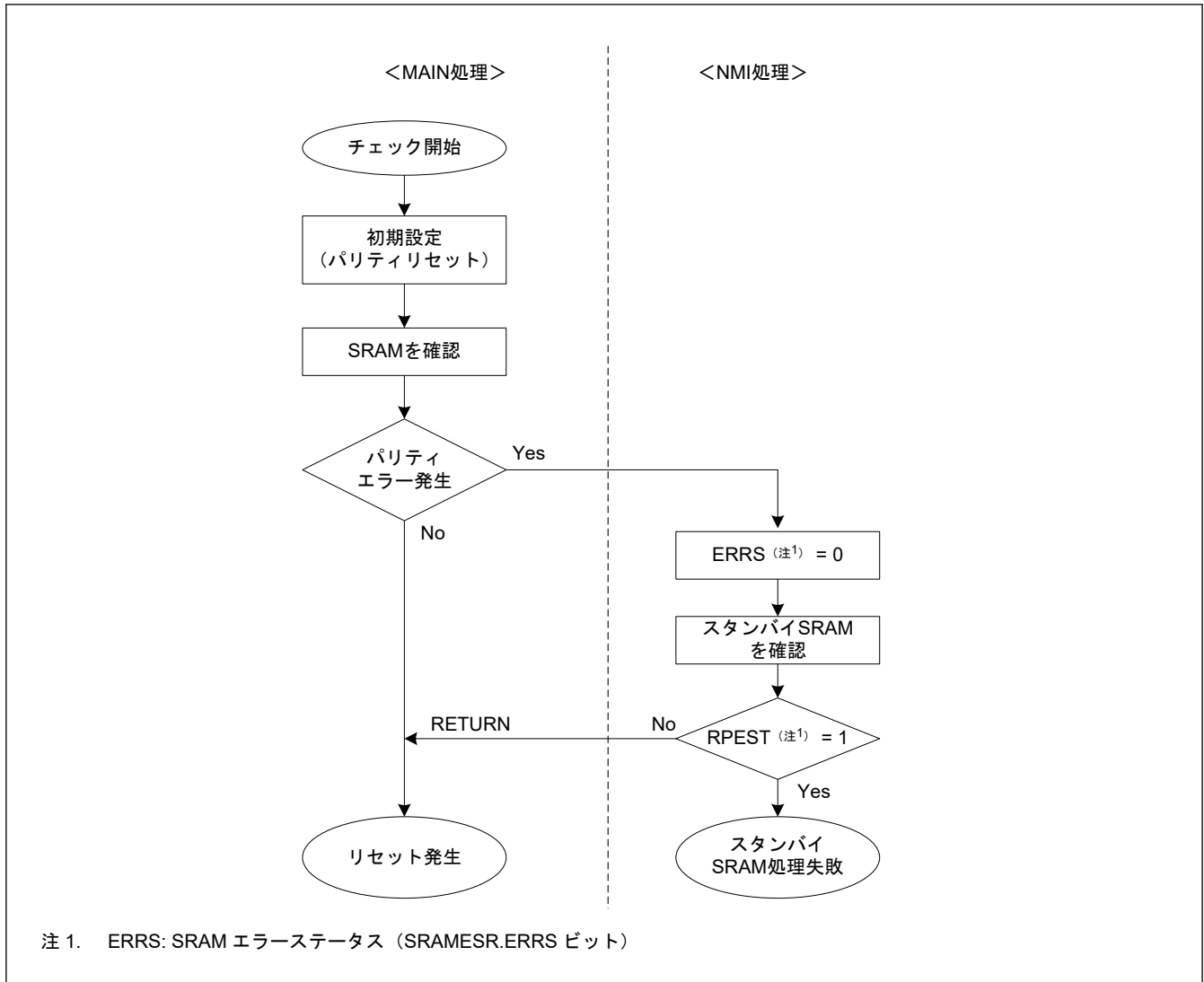
図 51.2 SRAM パリティ割り込み許可の場合のスタンバイ SRAM パリティチェックのフロー
