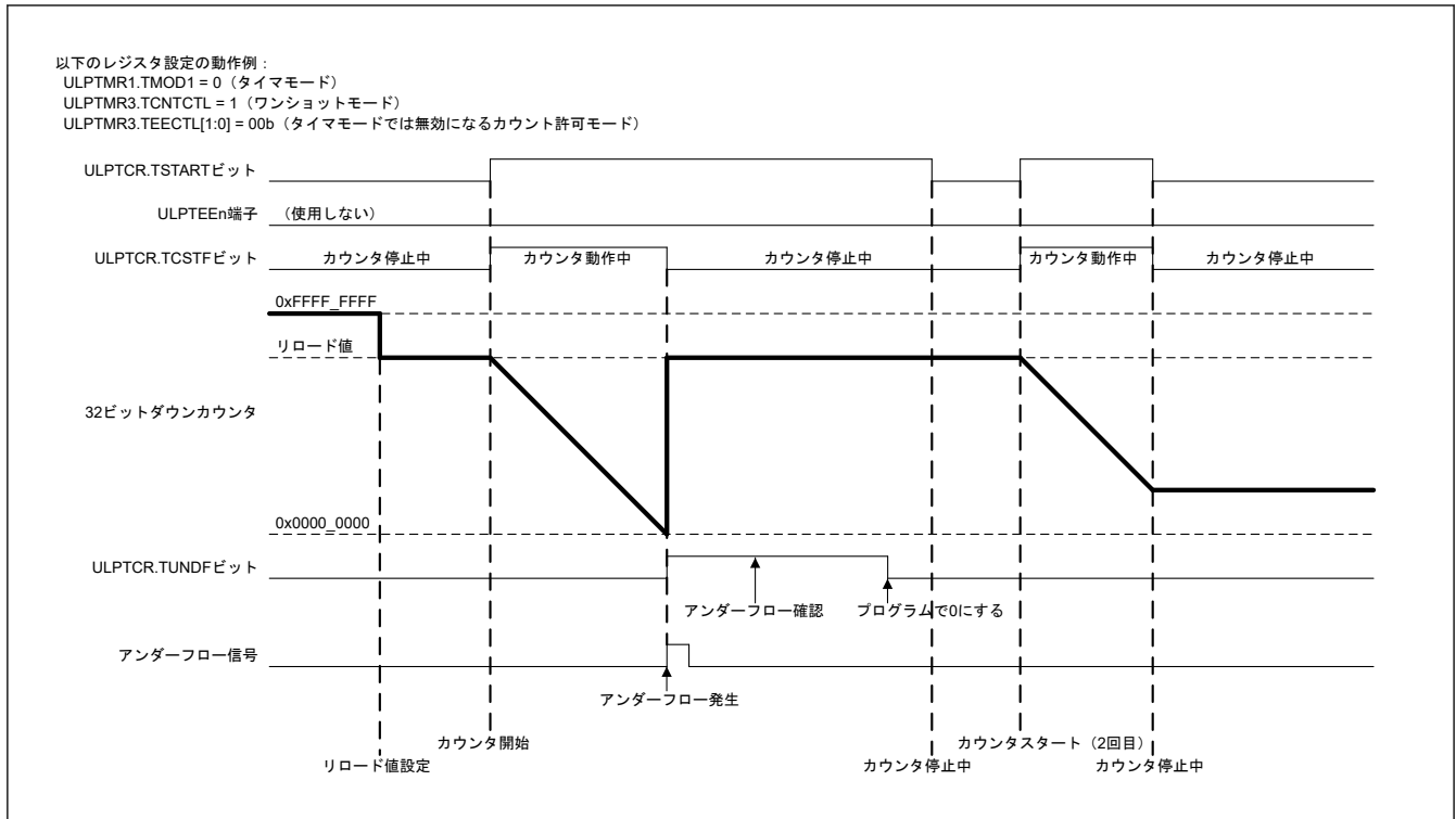
図 23.3 タイマ&ワンショットモードでの動作例
