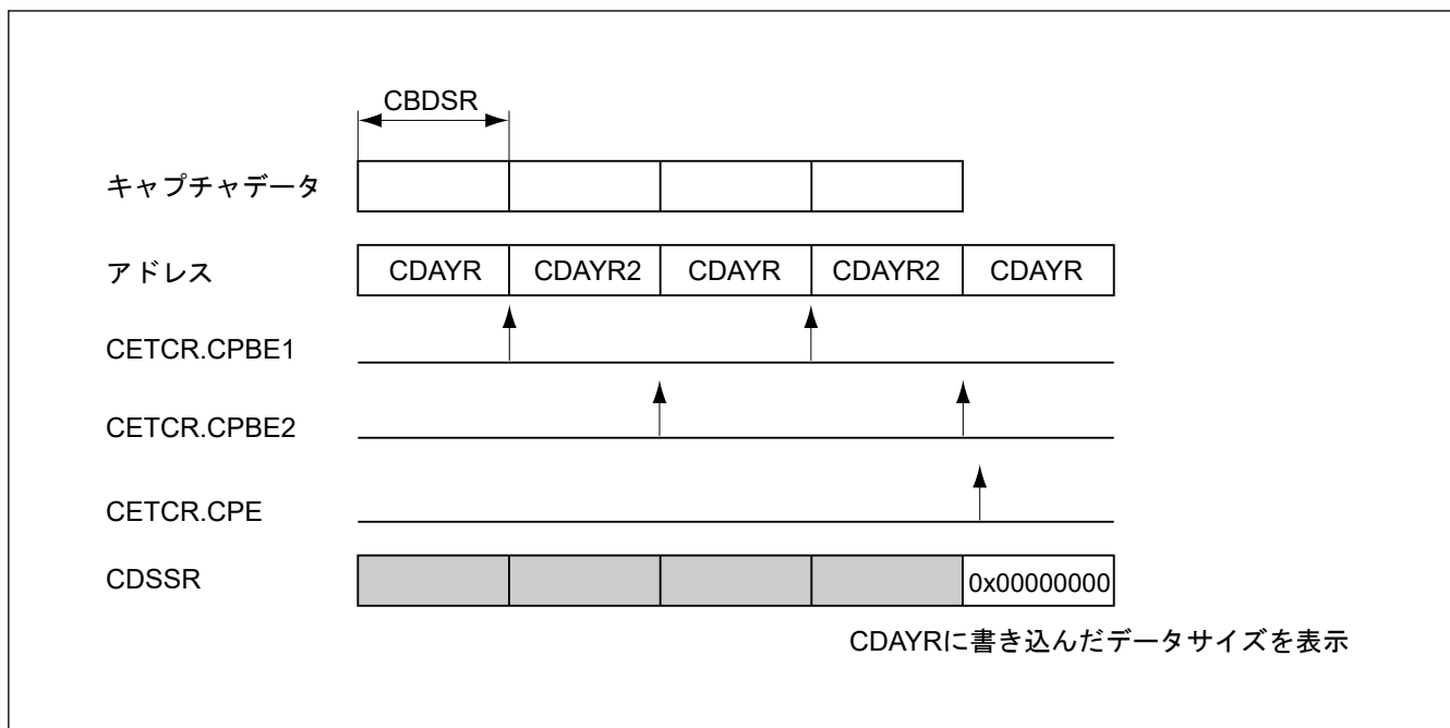
図 53.48 バンドル書き込み時の CDSSR 動作タイミングイメージ図 (バンドル書き込み終了とキャプチャ終了が同時の場合)
