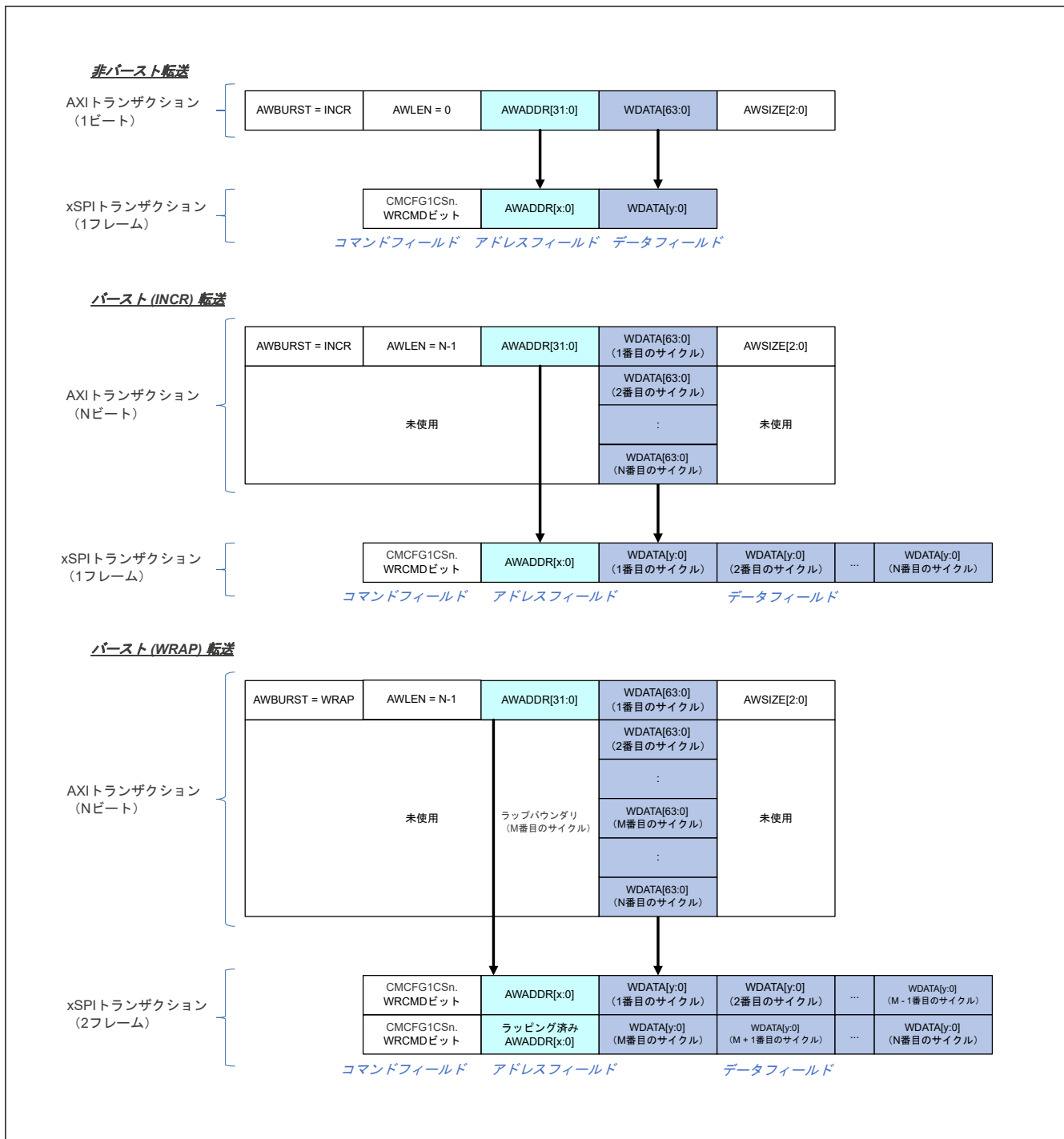
図 37.13 書き込みアクセス時の xSPI フレームのフォーマット (通常フォーマット)
