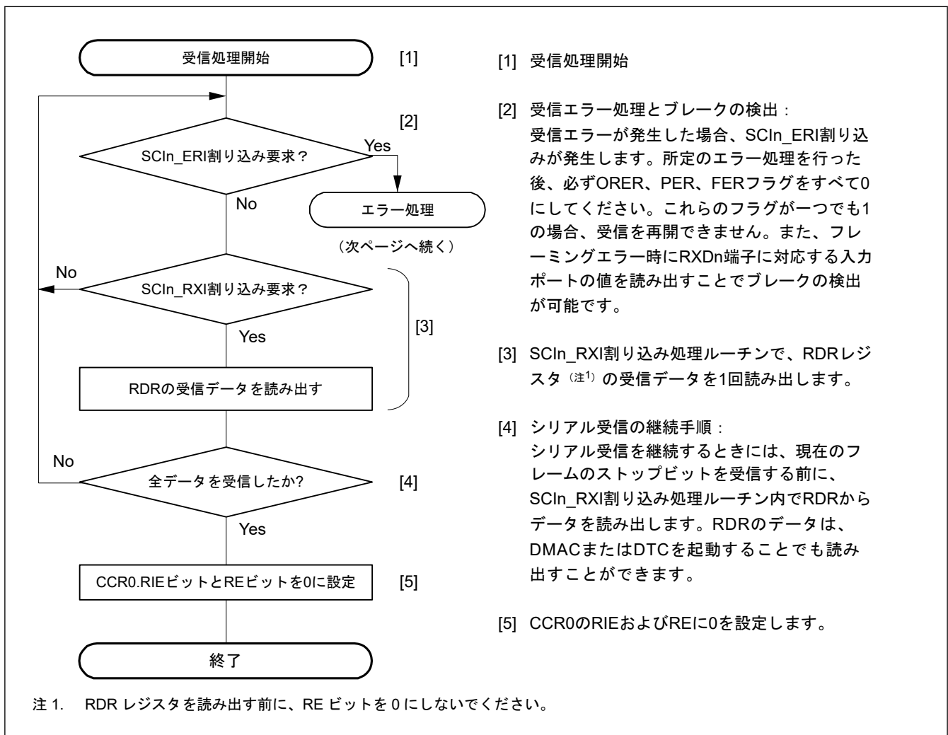
図 31.21 調歩同期式モードにおけるシリアル受信のフローチャート例 (非 FIFO 選択、アドレス一致検出無効時) (1)
