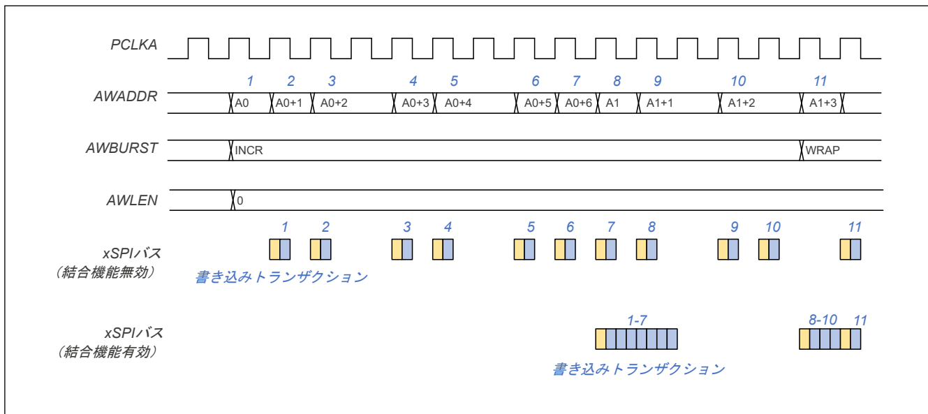
図 37.14 結合機能
