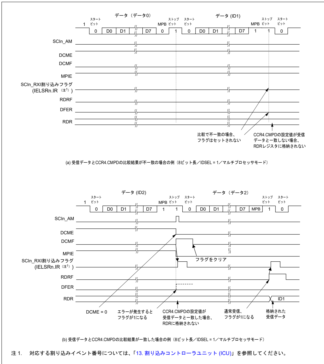
図 31.10 アドレス一致検出の例 (2) (マルチプロセッサモード)
