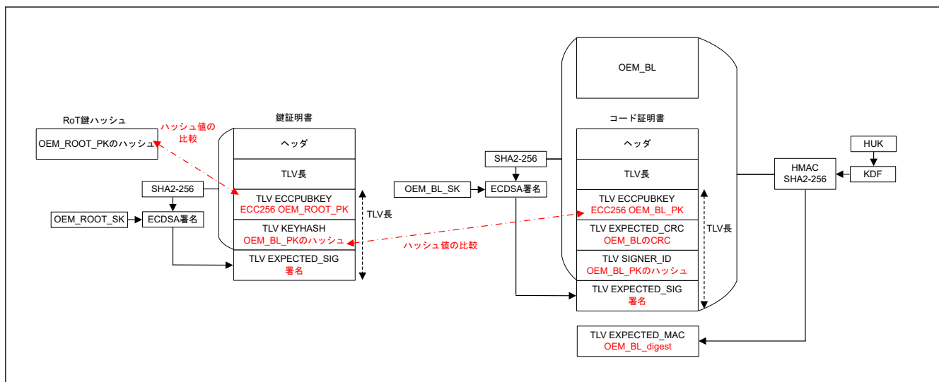
図 43.13 検証構成と証明書の形式
