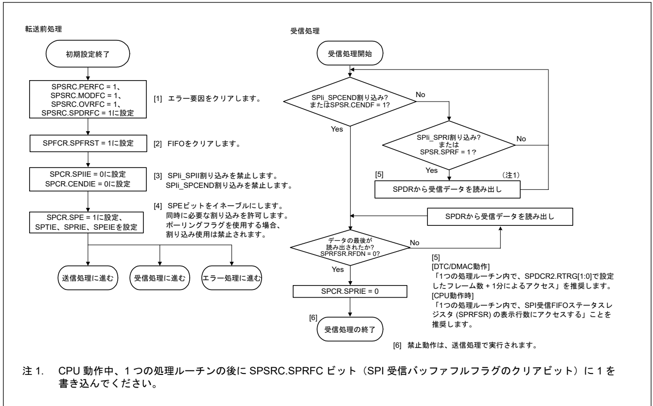
図 36.65 マスタモードでの受信手順
