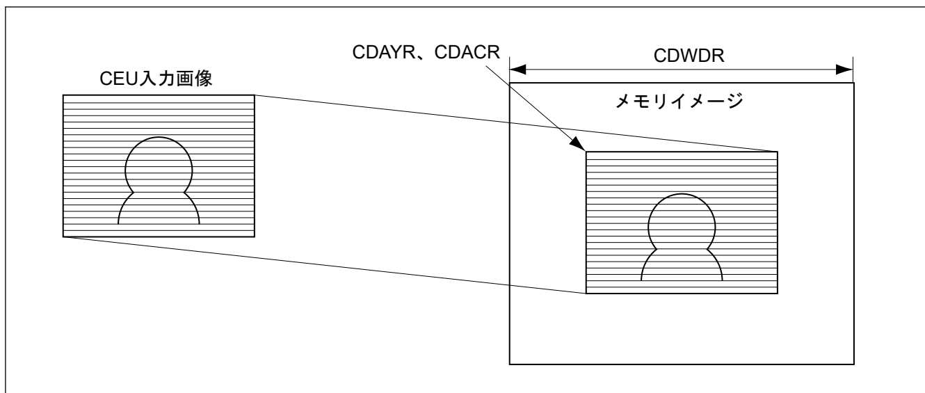
図 53.24 フレームキャプチャ画像および片フィールドキャプチャ画像のメモリ格納イメージ
