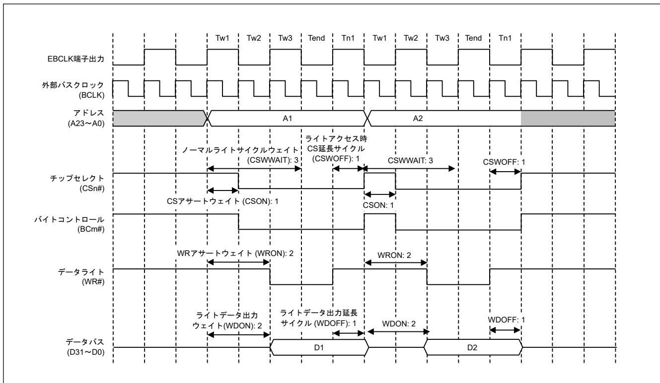
図 14.14 ノーマルライトアクセスの動作例 (EBCLK 端子出力選択ビットで BCLK の 2 分周を設定した場合、および 1 転送要求に対して 2 回バスアクセスが発生する場合) (n = 0~7, m = 0~3)
