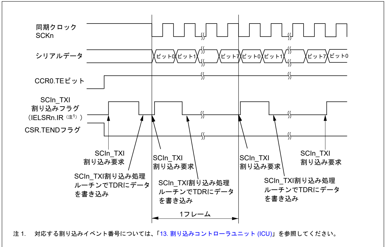
図 31.62 クロック同期式モードにおけるシリアル送信の動作例 (送信開始時に CTS 機能を使用しない場合)
