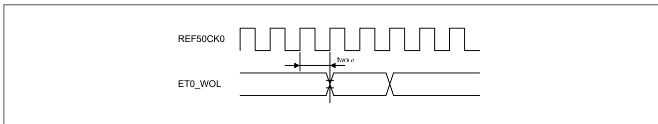
図 55.95 RMII に対する WOL 出カタイミング
