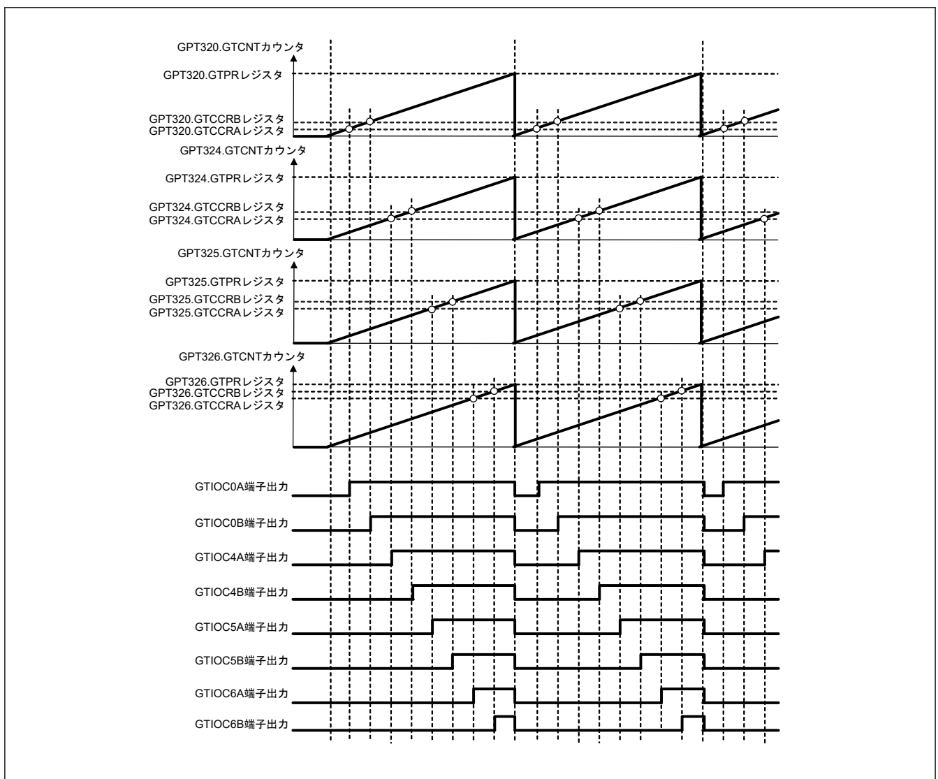
図 21.44 同期 PWM 出力例
