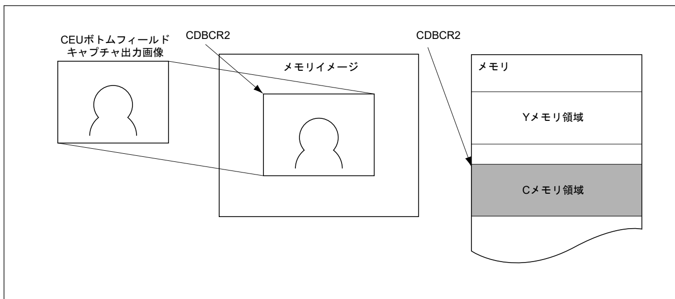
図 53.54 ボトムフィールドキャプチャ画像と色差成分メモリ領域の関係
