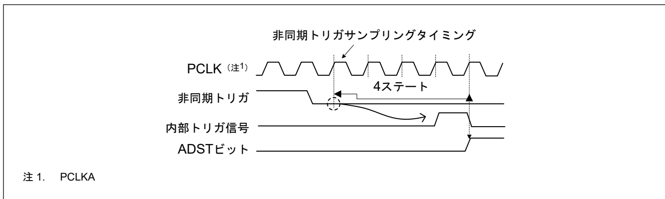
図 45.41 非同期トリガ入力タイミング
