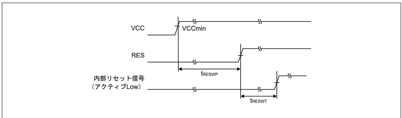
図 55.22 VCC が V POR 電圧しきい値を超える条件下での RES 端子入力タイミング
