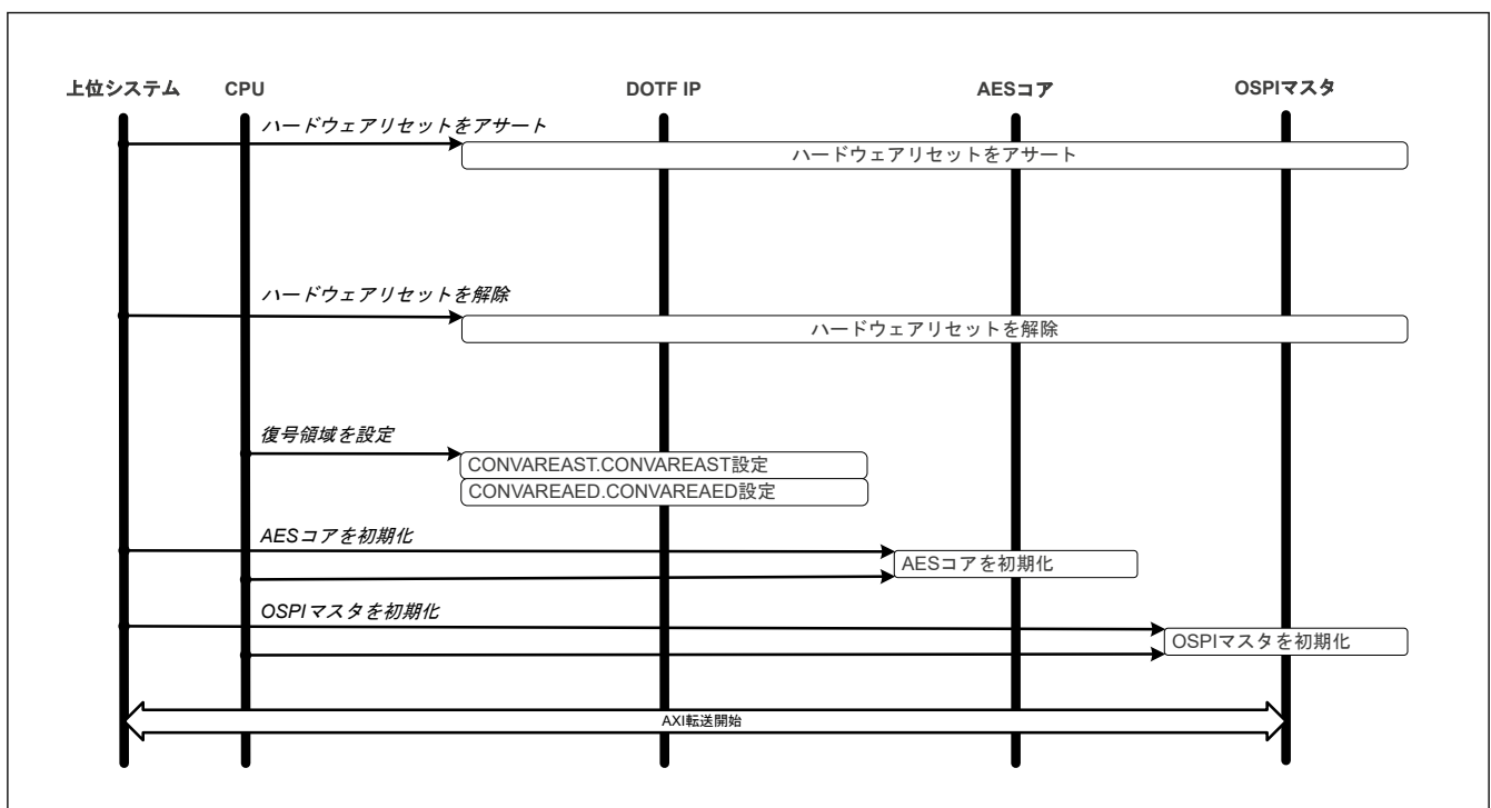
図 38.3 初期化フロー
