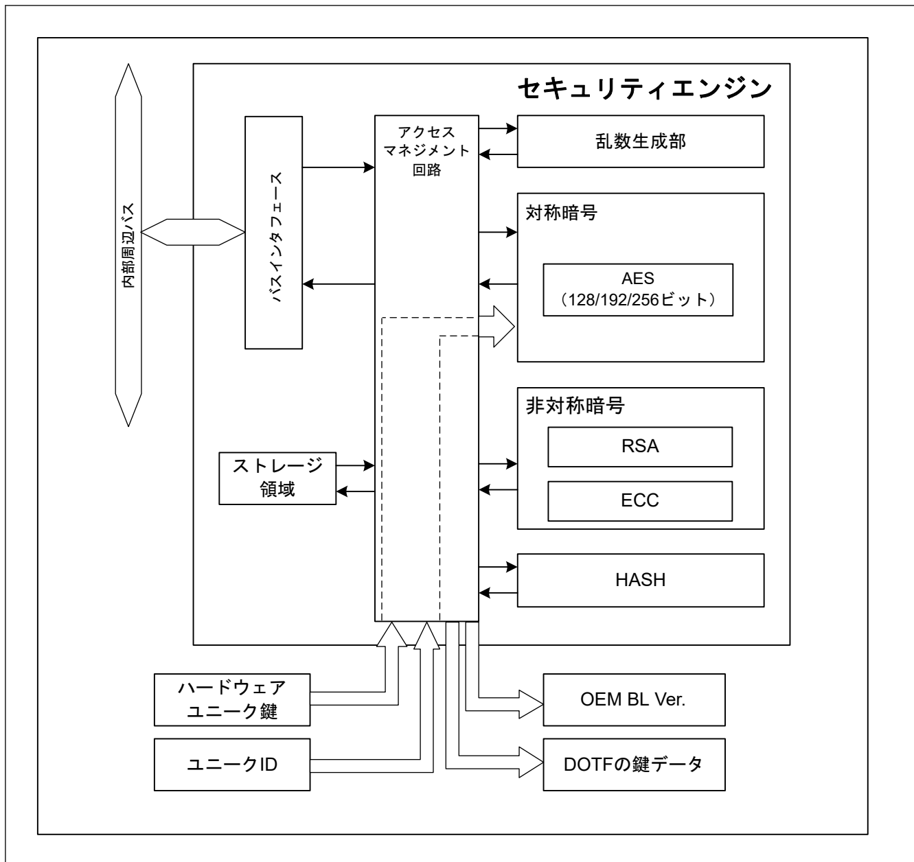
図 44.1 セキュリティエンジンのブロック図
