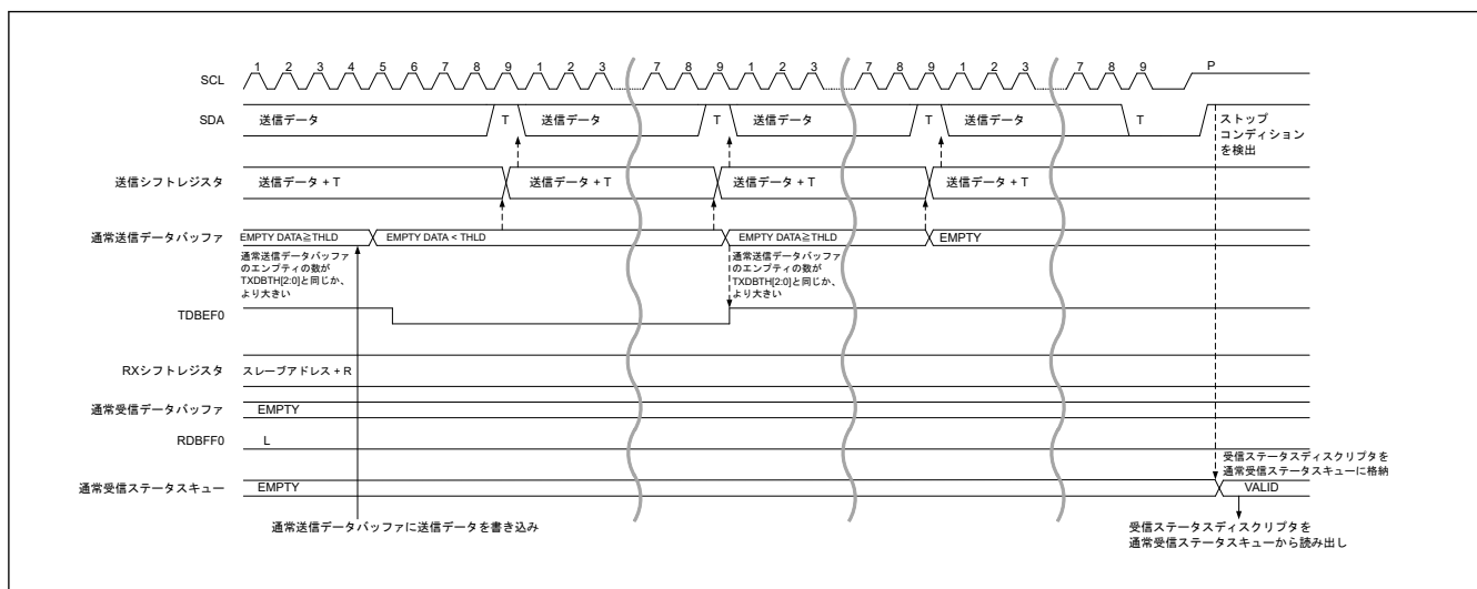
図 33.50 SDR データ読み出し転送タイミング (2/2)
