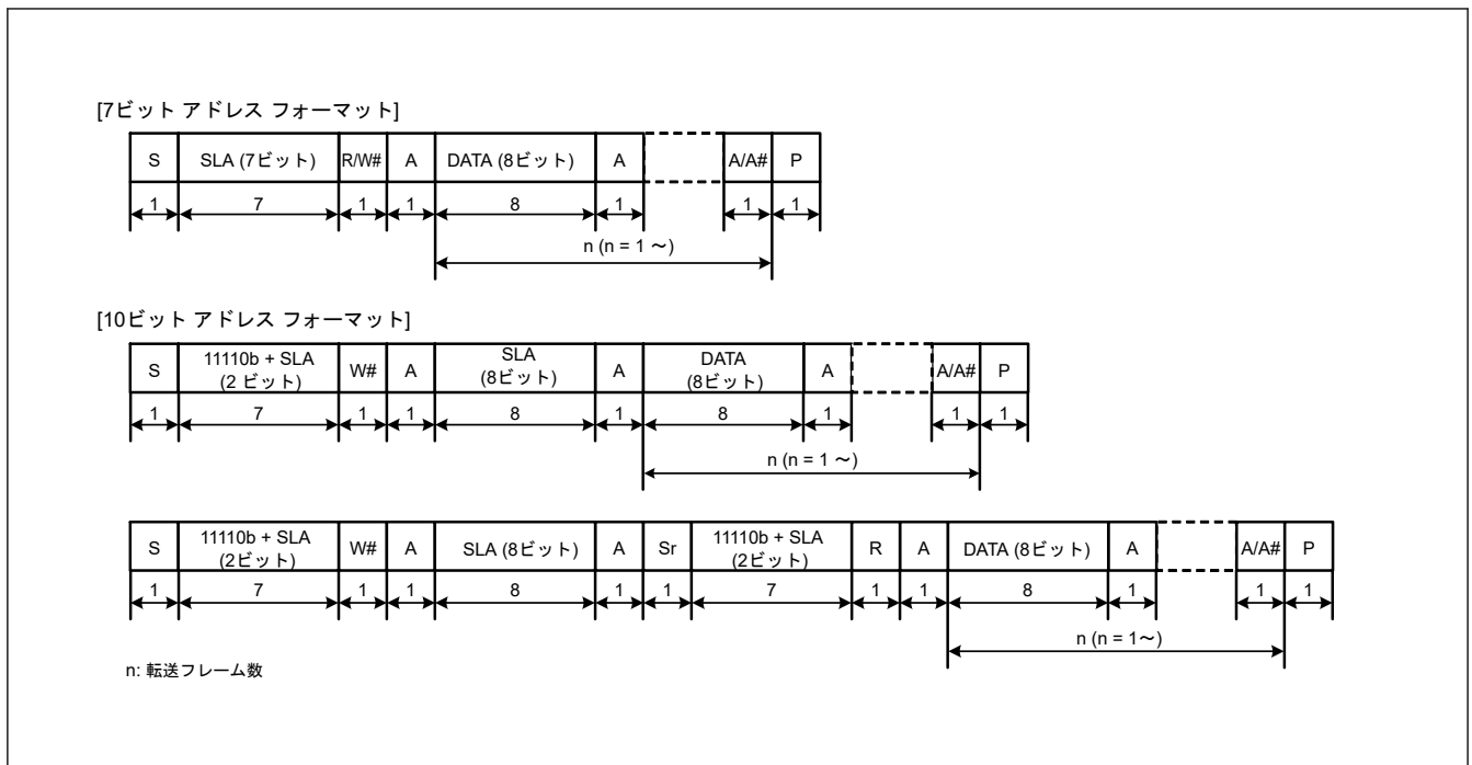
図 32.3 I2C パスフォーマット
