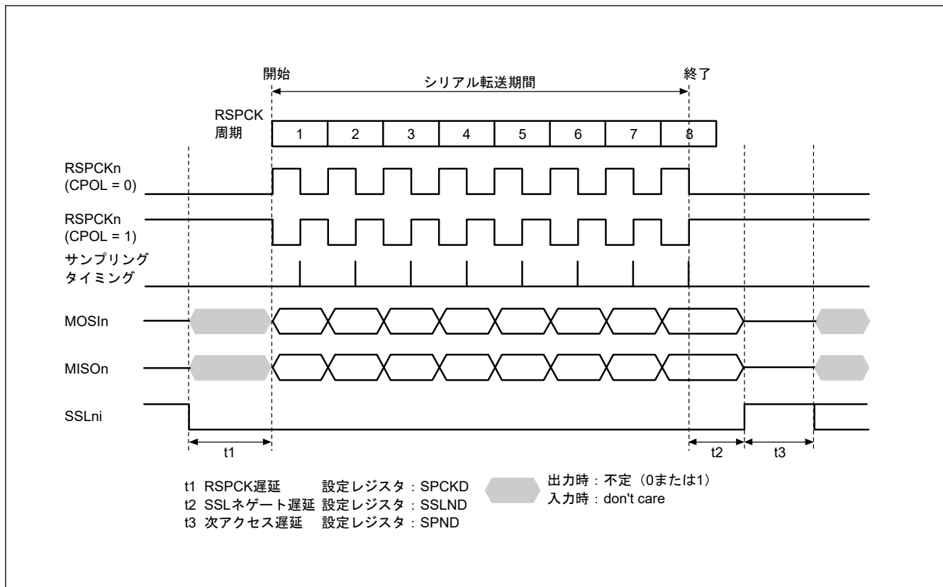
図 36.28 CPHA = 1、SPFRF = 0 の場合の SPI 転送フォーマット
