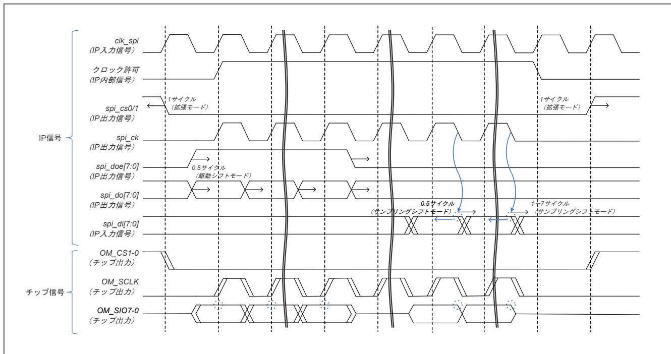
図 37.8 OM_DQS なし SDR のタイミング制御
