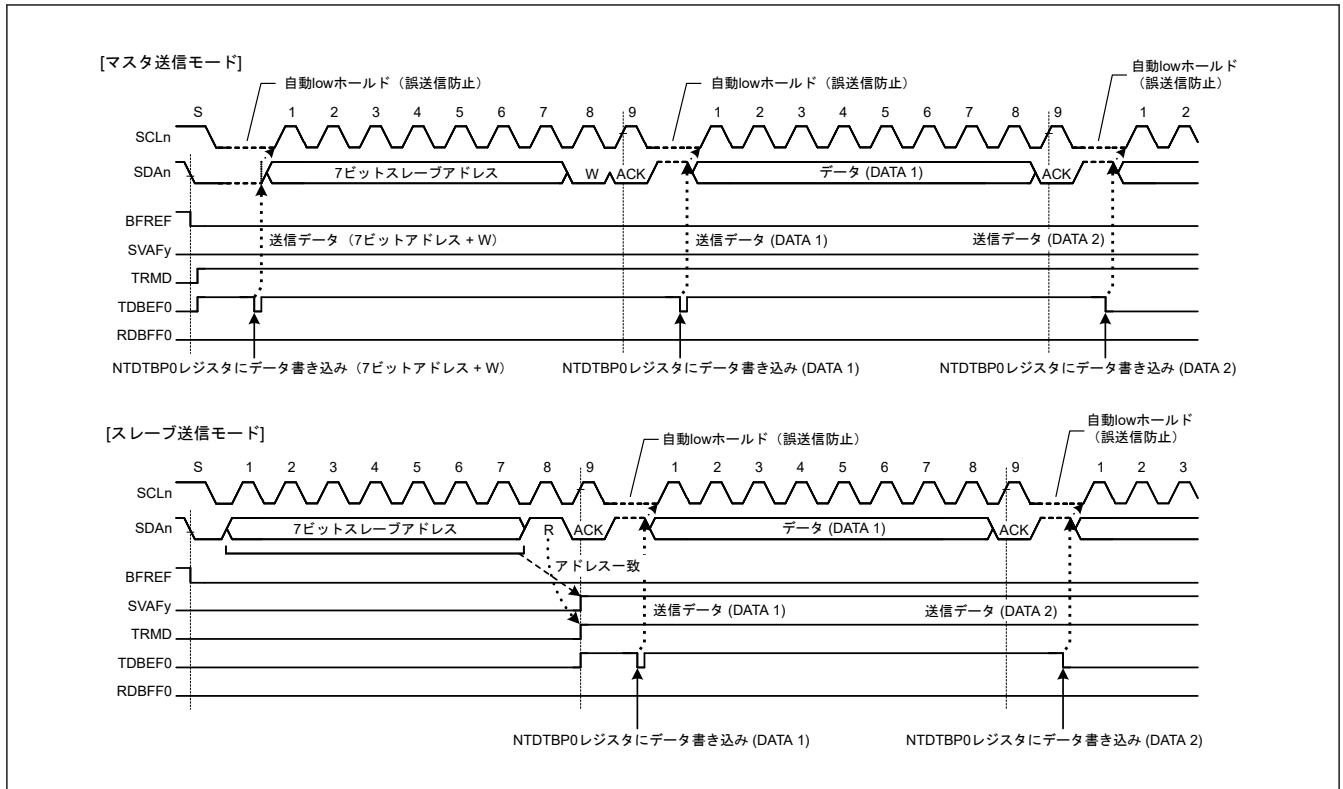
図 33.93 送信モード時の自動 Low ホールド動作
