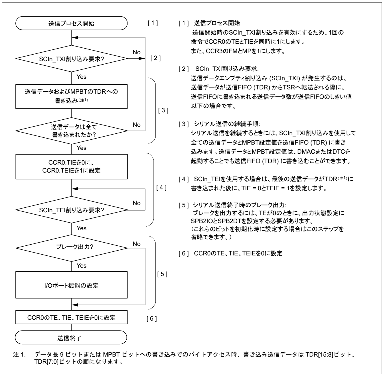
図 31.38 マルチプロセッサモードにおけるシリアル送信のフローチャート例 (FIFO 選択時)
