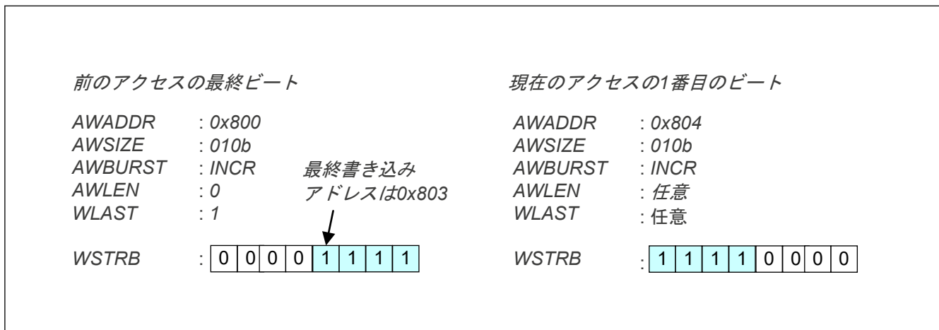
図 37.15 AXI アクセスでのデータ結合例
