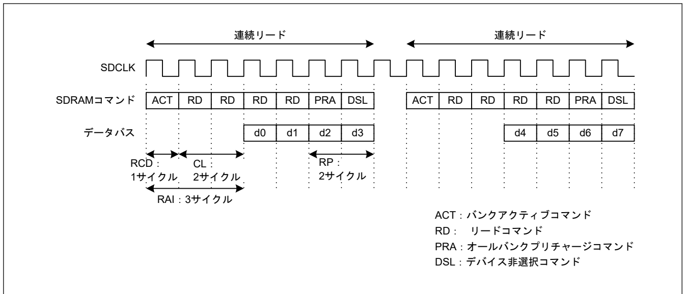
図 14.62 連続リードタイミング例 (1)
