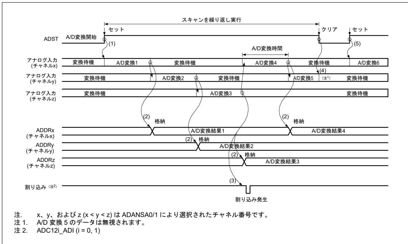
図 45.17 連続スキャンモードの基本動作例（アナログ入力（チャンネル x~z）選択）
