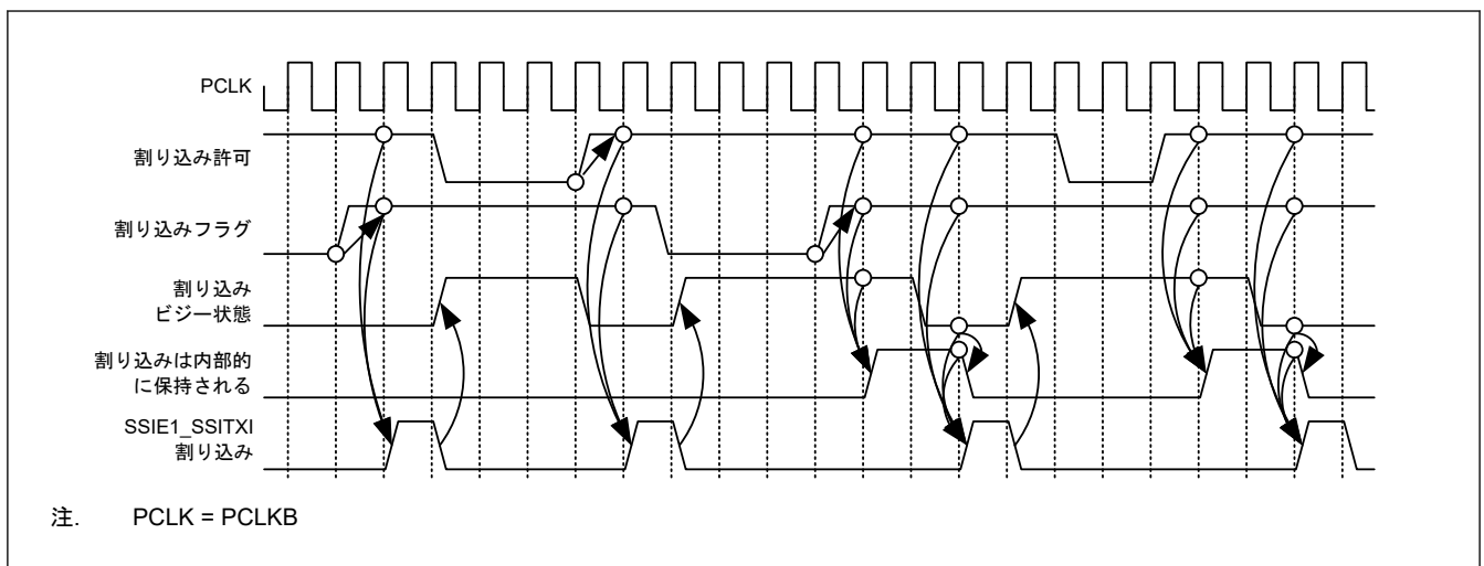
図 39.60 SSIE1_SSITXI 割り込みタイミング図
