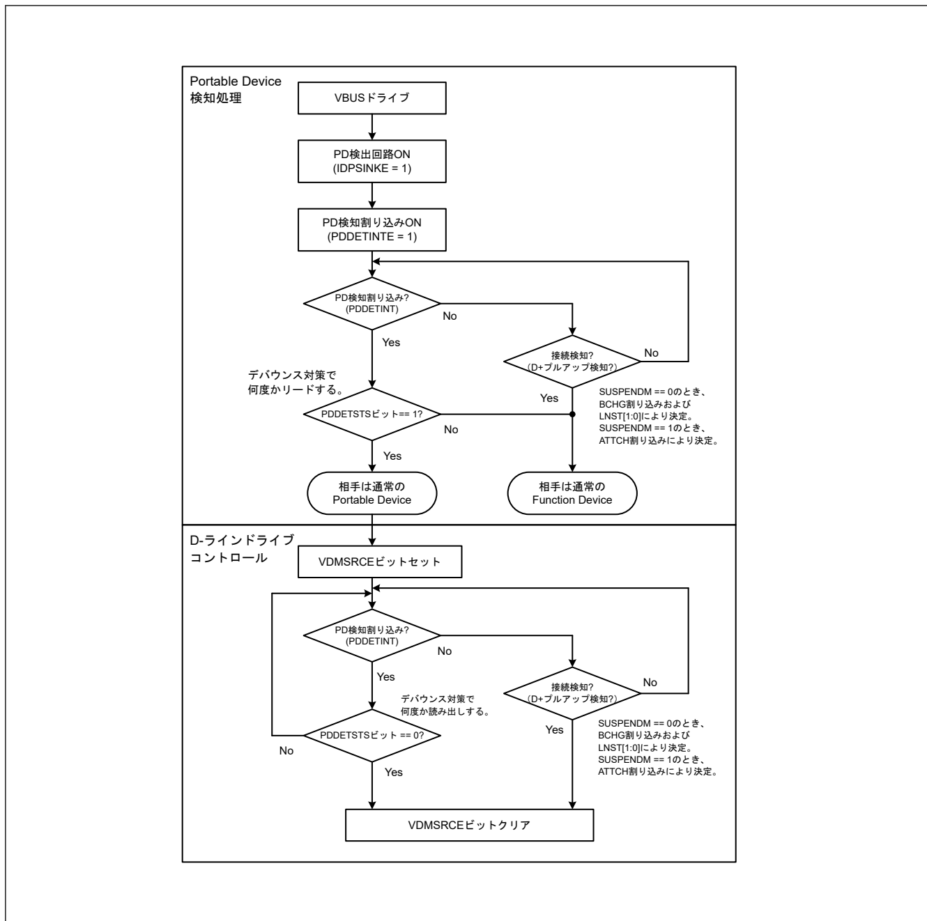
図 30.21 ハードウェアに Portable Device 検出機能搭載時の Charging Downstream ポート処理フロー
