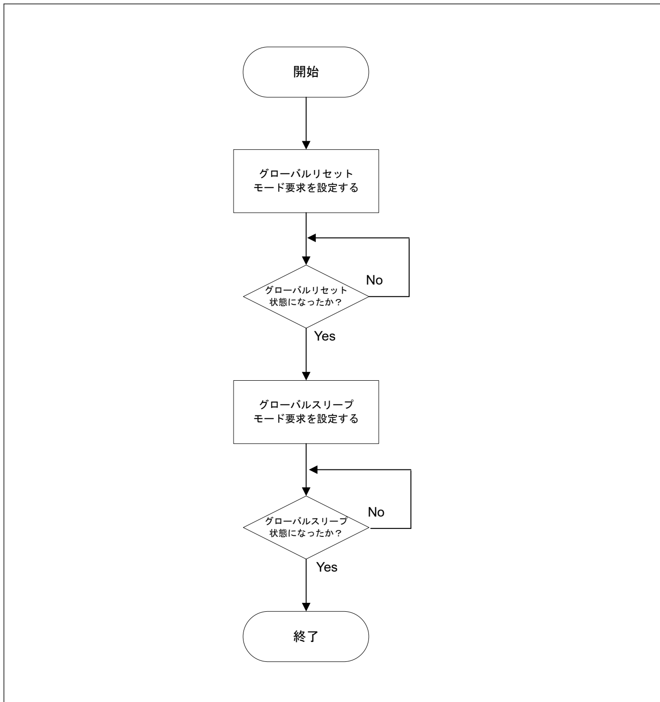
図 34.3 グローバルスリープモードへの遷移手順
