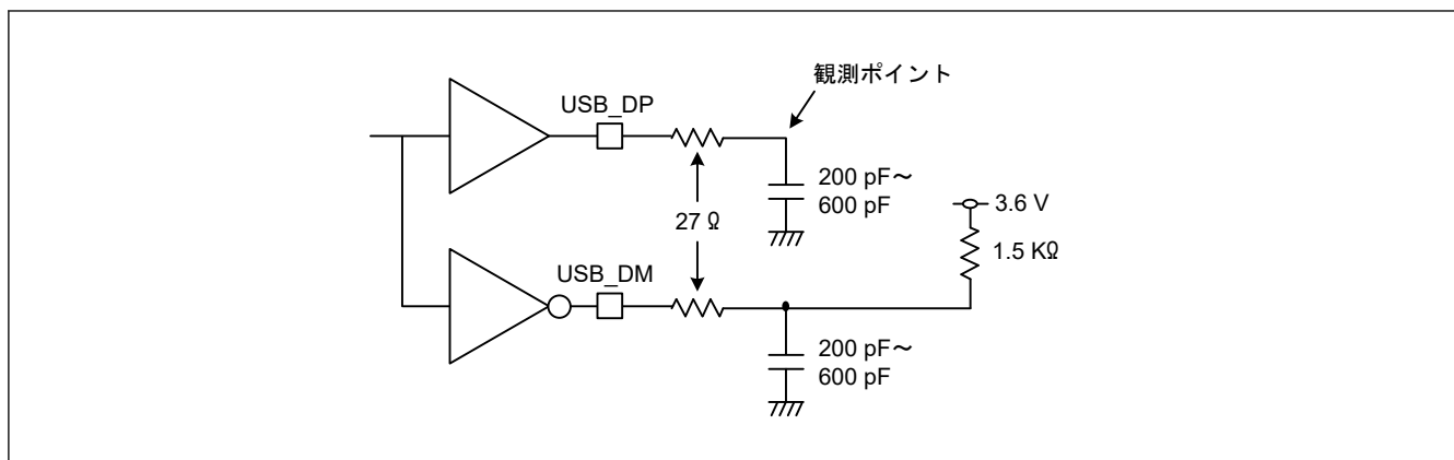
図 55.109 Low-speed モードにおける測定回路
