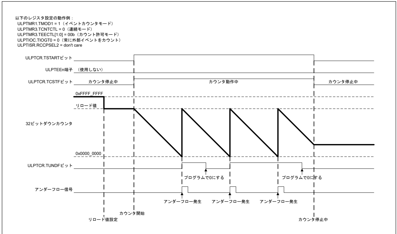
図 23.4 イベントカウンタ&連続&カウント許可モードの動作例 (ULPTIOC.TIOGT0 ビットが 0 の場合)
