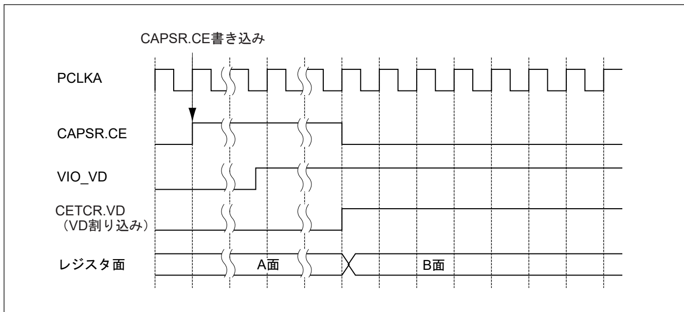
図 53.2 レジスタ面切り替えタイミング (データイネーブル取り込みモードかつ VD 正極性の場合)
