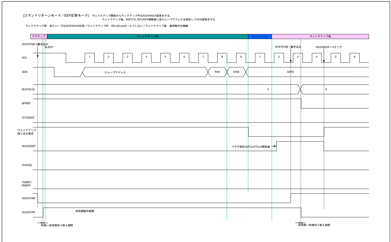
図 33.133 コマンドリカバリモードと EEP 応答モードのタイミング
