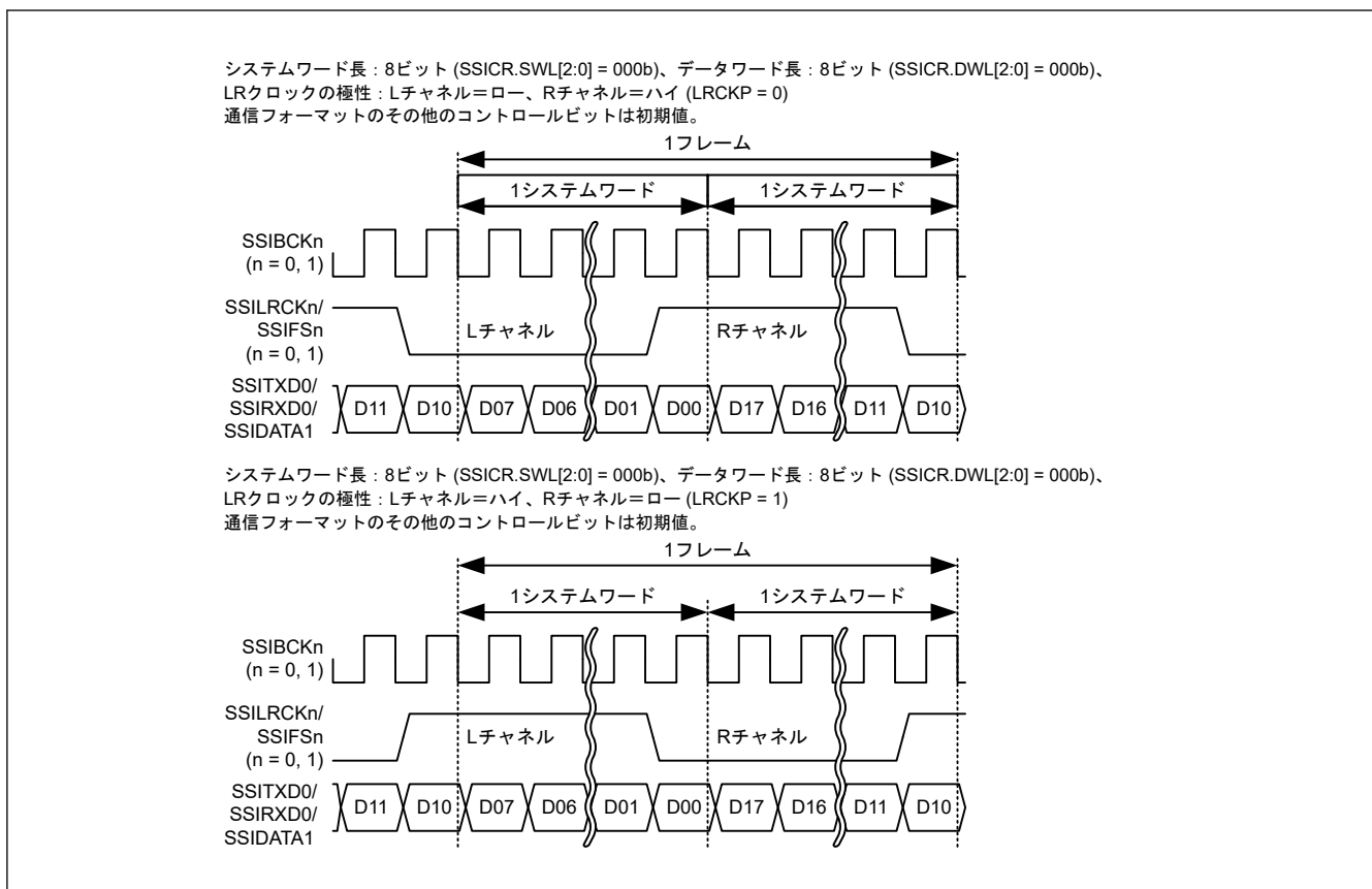
図 39.12 LR クロック/フレーム同期極性設定
