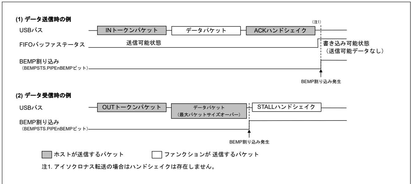
図 29.13 デバイスコントローラモード時の BEMP 割り込み発生タイミング
