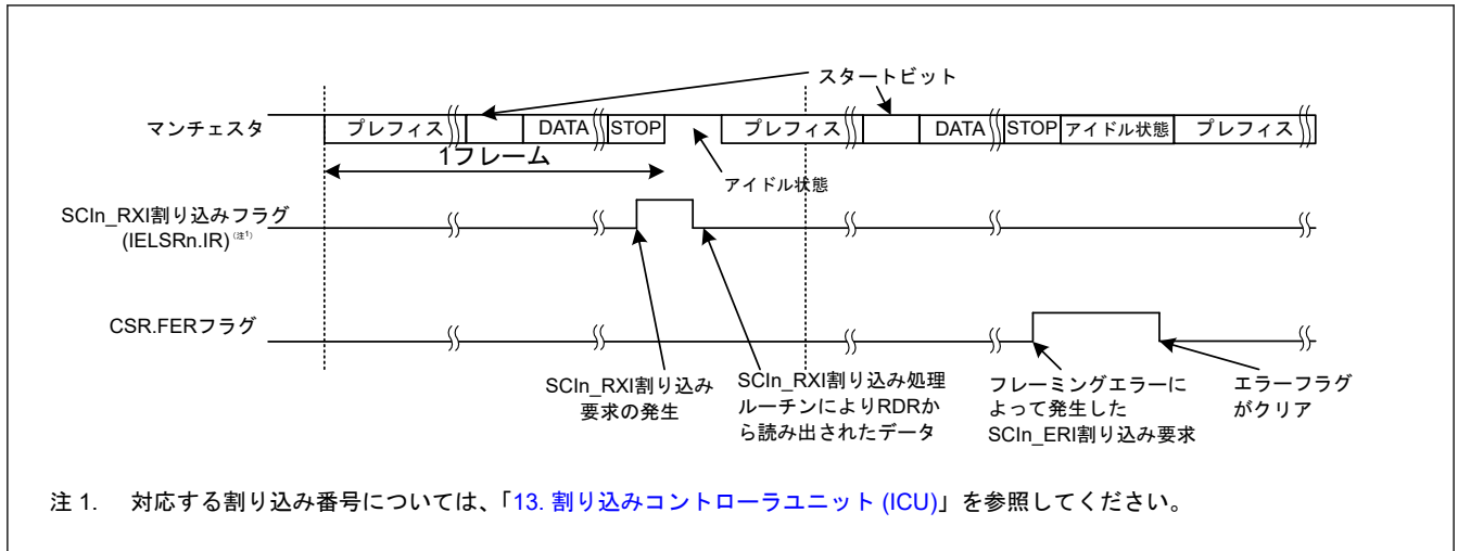
図 31.56 マンチェスタモードにおけるシリアルデータ受信の動作例（プレフィスあり）
