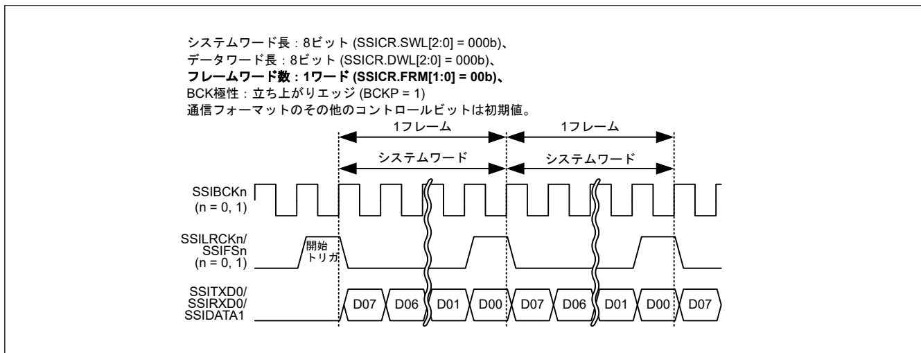
図 39.38 モノラルフォーマットにおけるショートフレーム（パディングなし、システムワード長 = データワード長）
