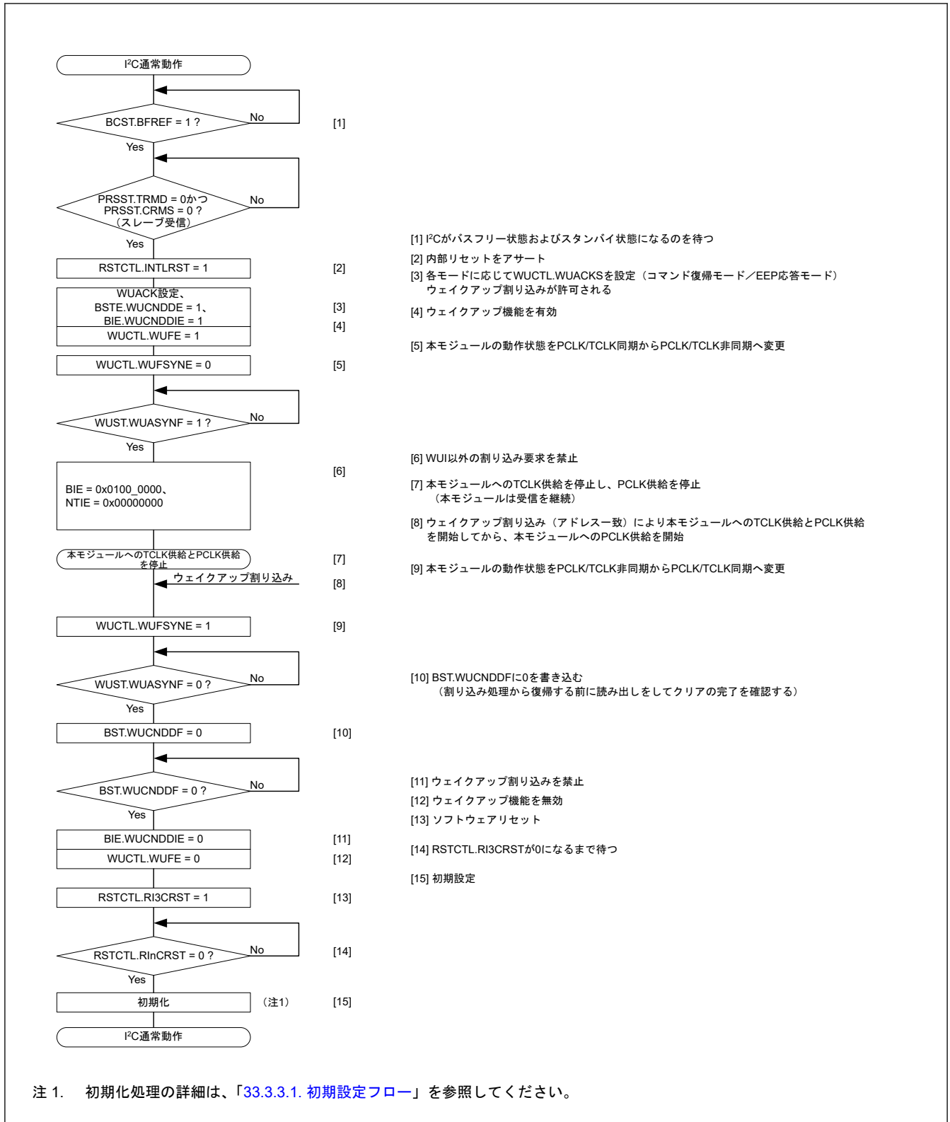
図 33.131 コマンドリカバリモードと EEP 応答モードの使用例 (スレープアドレス一致に起因するウェイクアップ割り込みによるウェイクアップリカバリの場合)
