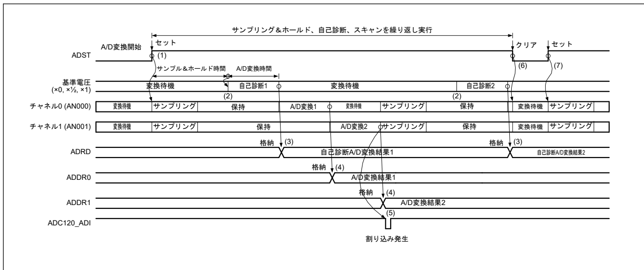
図 45.21 連続スキャンモードの動作例（チャンネル専用サンプル&ホールド回路使用、AN000 および AN001 選択+自己診断）
