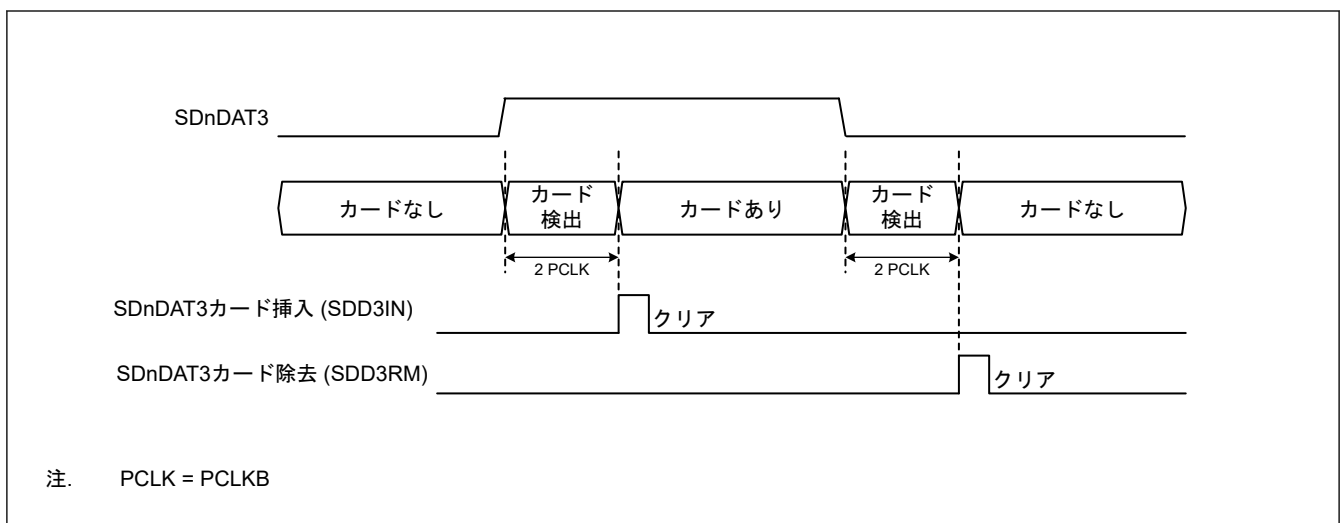
図 40.8 SDnDAT3 による SD カード検出
