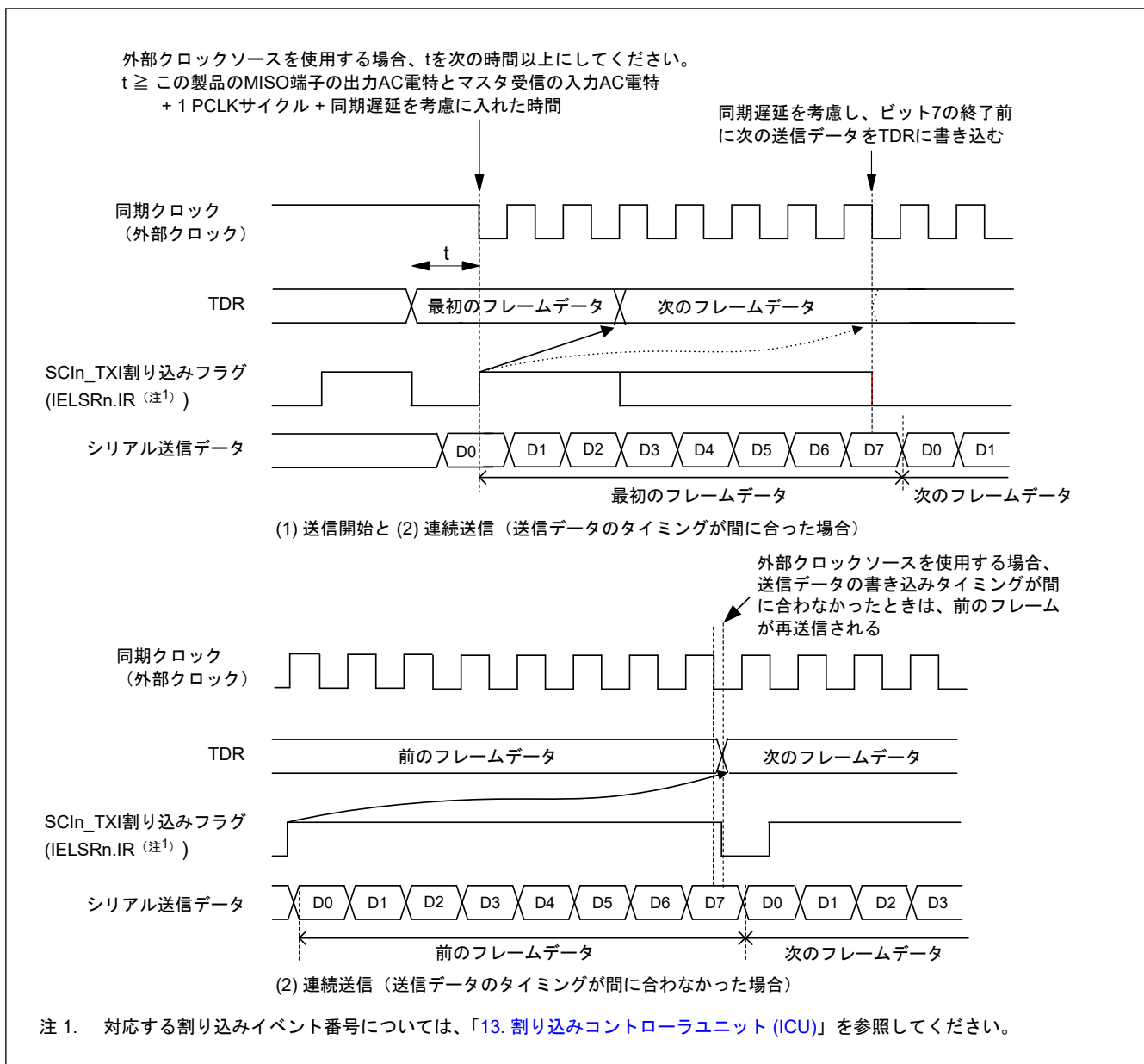
図 31.121 クロック同期式送信時の外部クロック使用に関する制約事項
