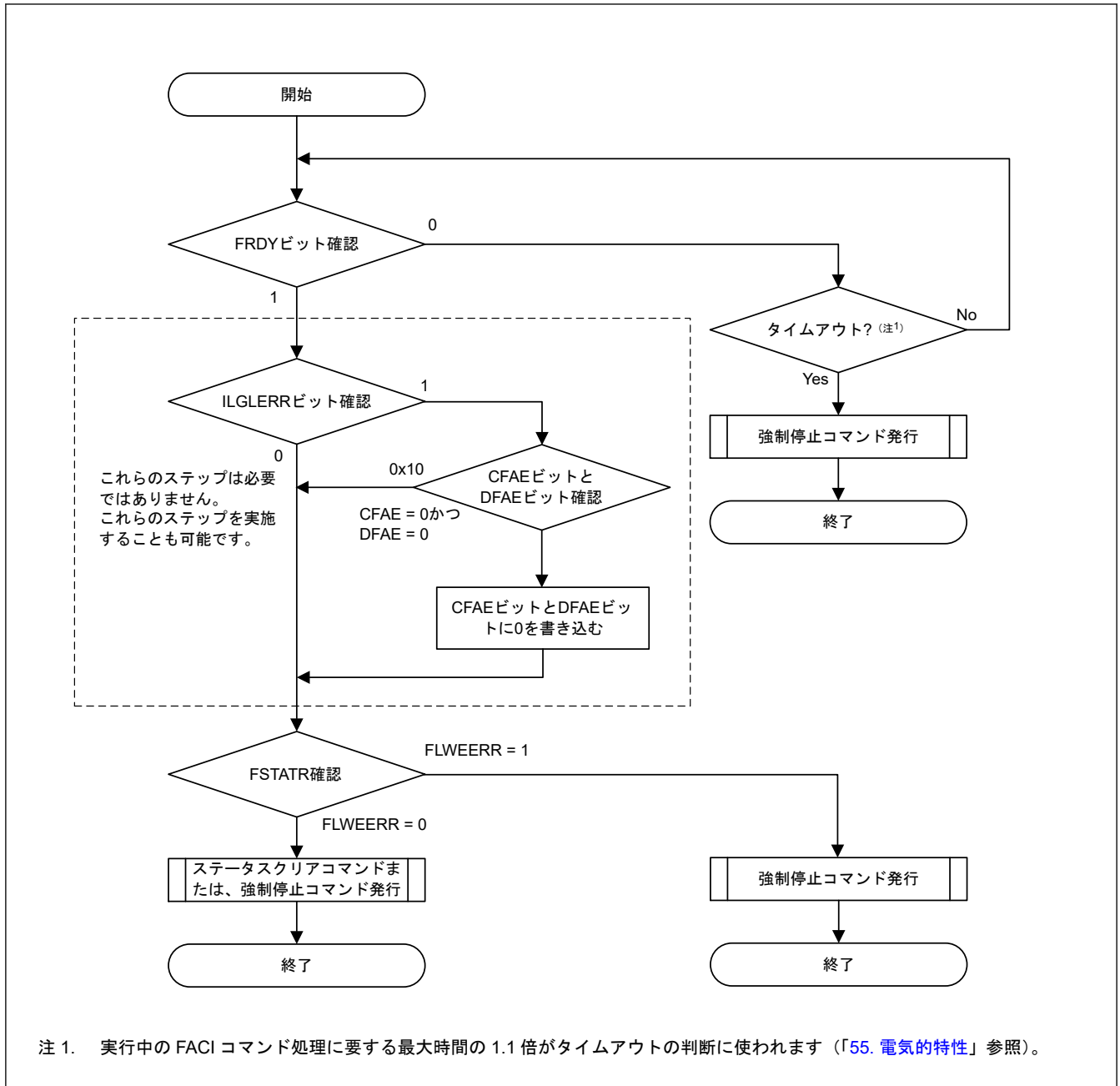
図 52.13 コマンドロック状態からの復帰フロー
