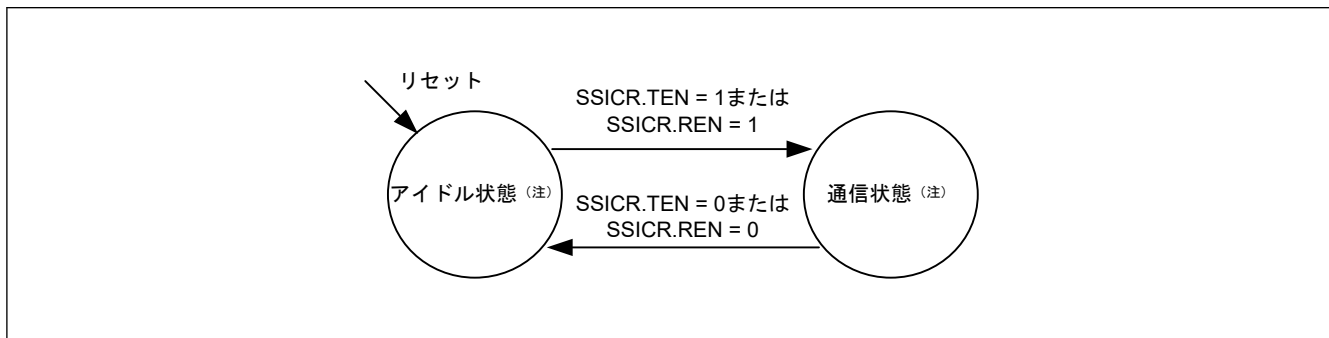
図 39.43 SSIE の状態遷移
