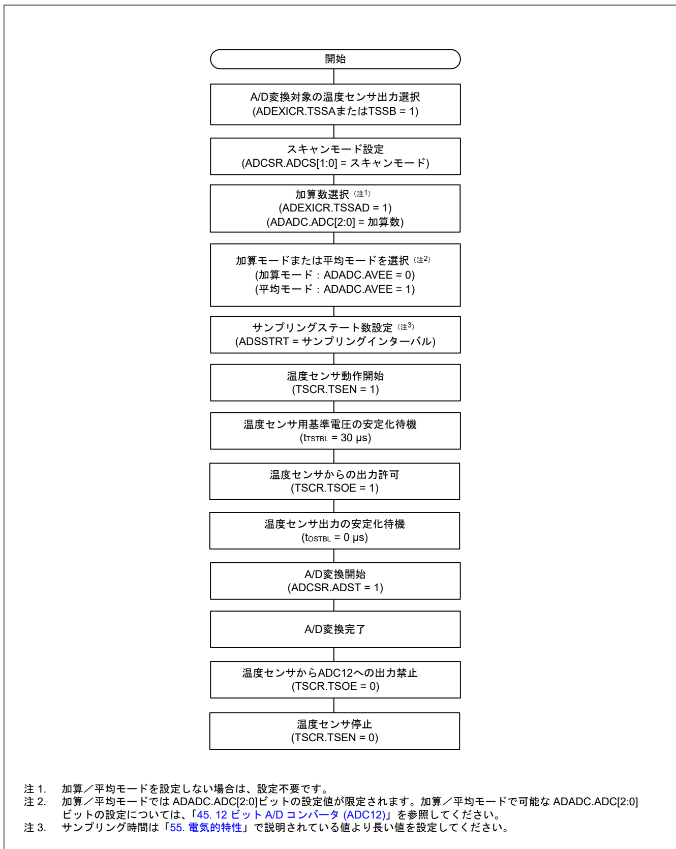
図 47.2 TSN の使用手順例
