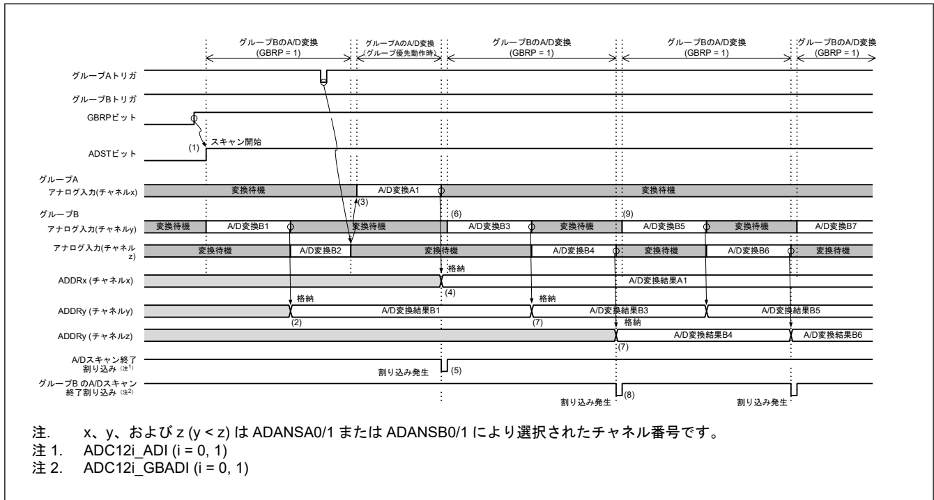
図 45.31 グループ優先動作の例 1-5 : グループ B のシングルスキャン連続動作 (ADGSPCR.GBRP = 1, ADGSPCR.LGRRS = 0 の場合)
