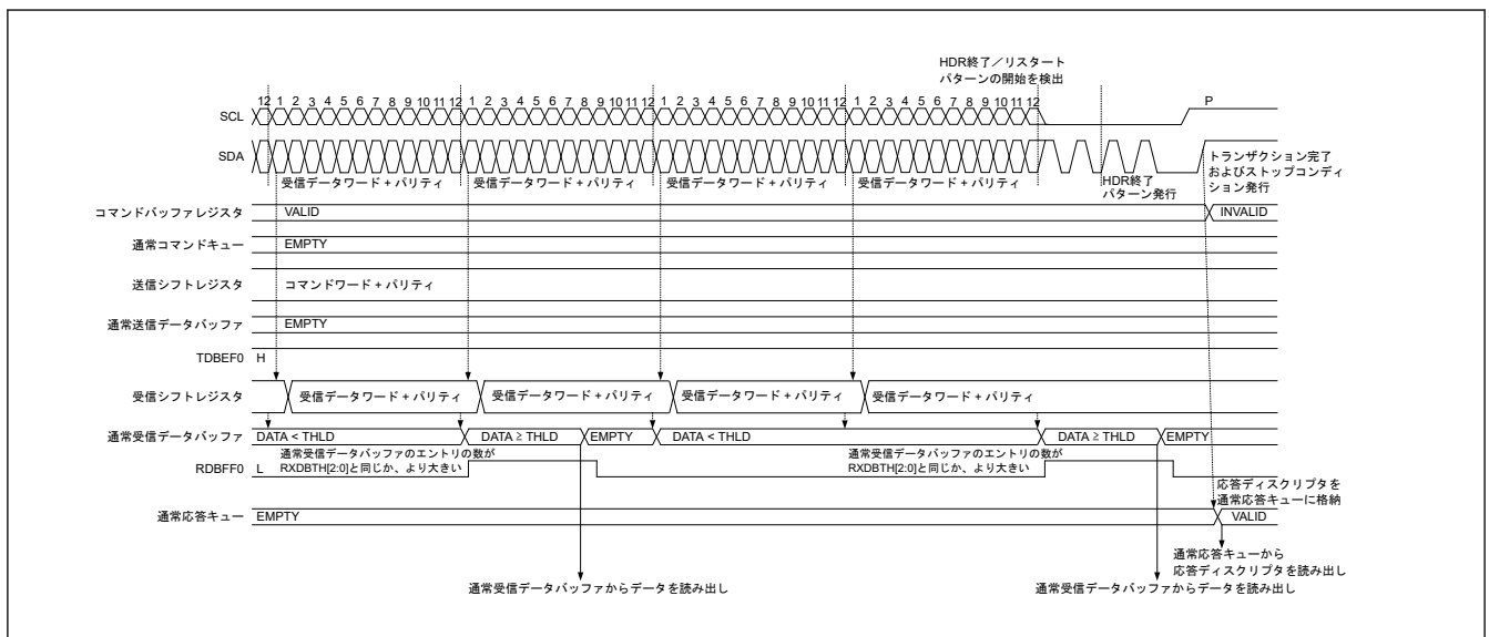
図 33.33 HDR データ読み出し転送 (HDR-TSP、TSL) タイミング (2/2)
