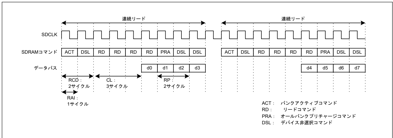
図 14.64 連続リードタイミング例 (3)
