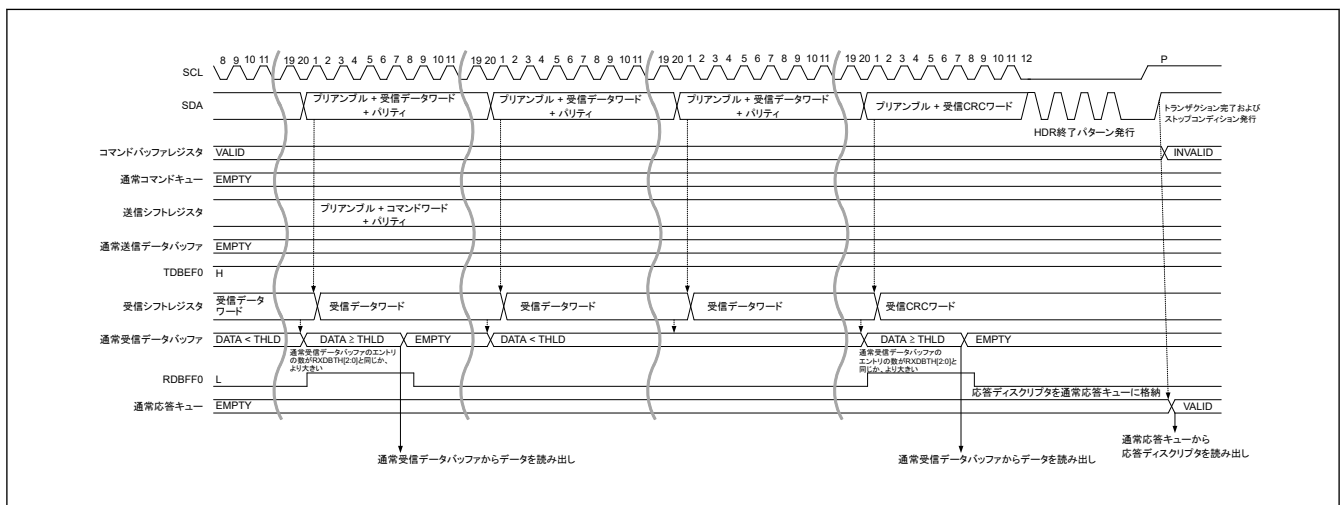
図 33.31 HDR データ読み出し転送 (HDR-DDR) タイミング (2/2)
