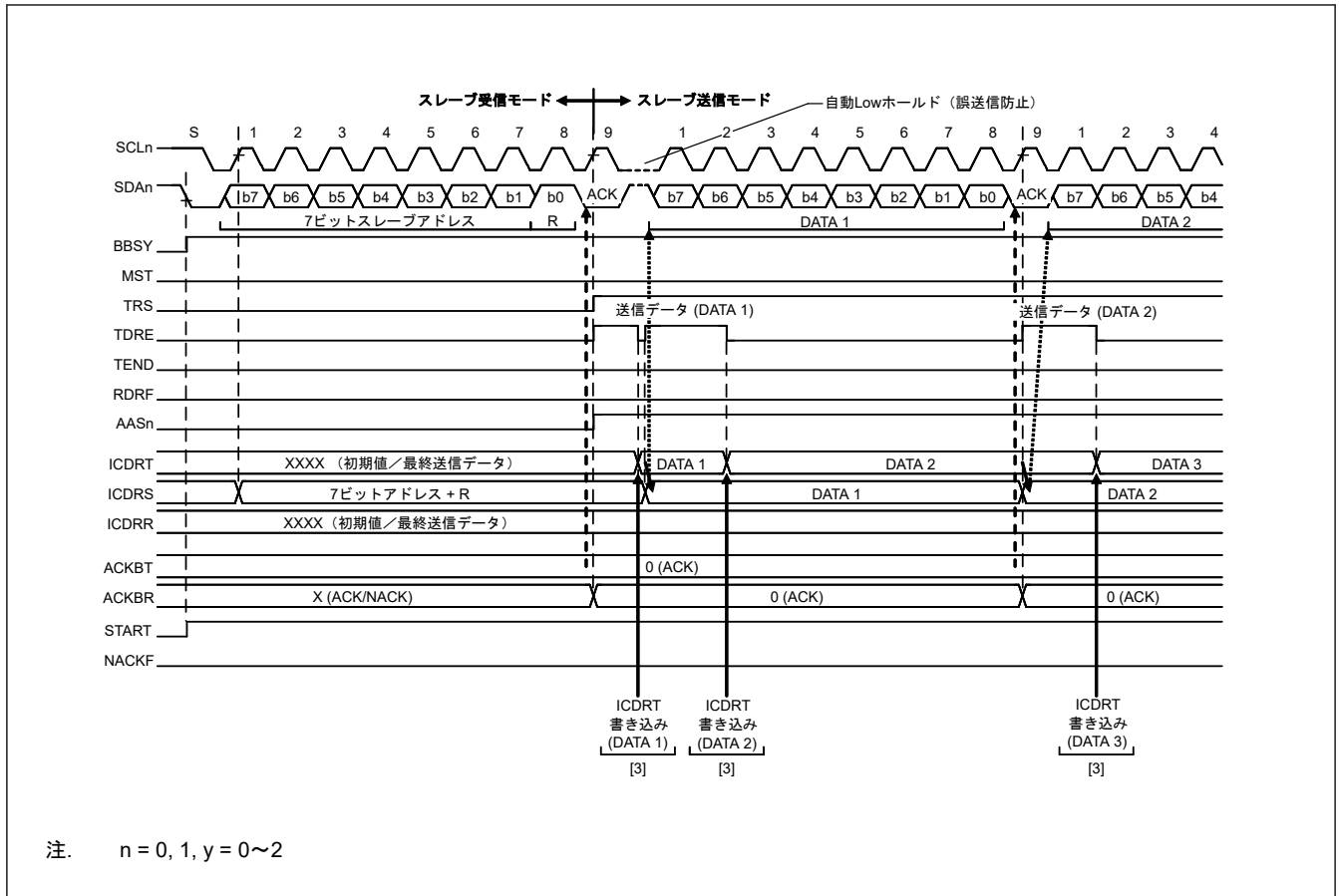
図 32.16 スレーブ送信の動作タイミング (1) (7ビットアドレスフォーマット)
