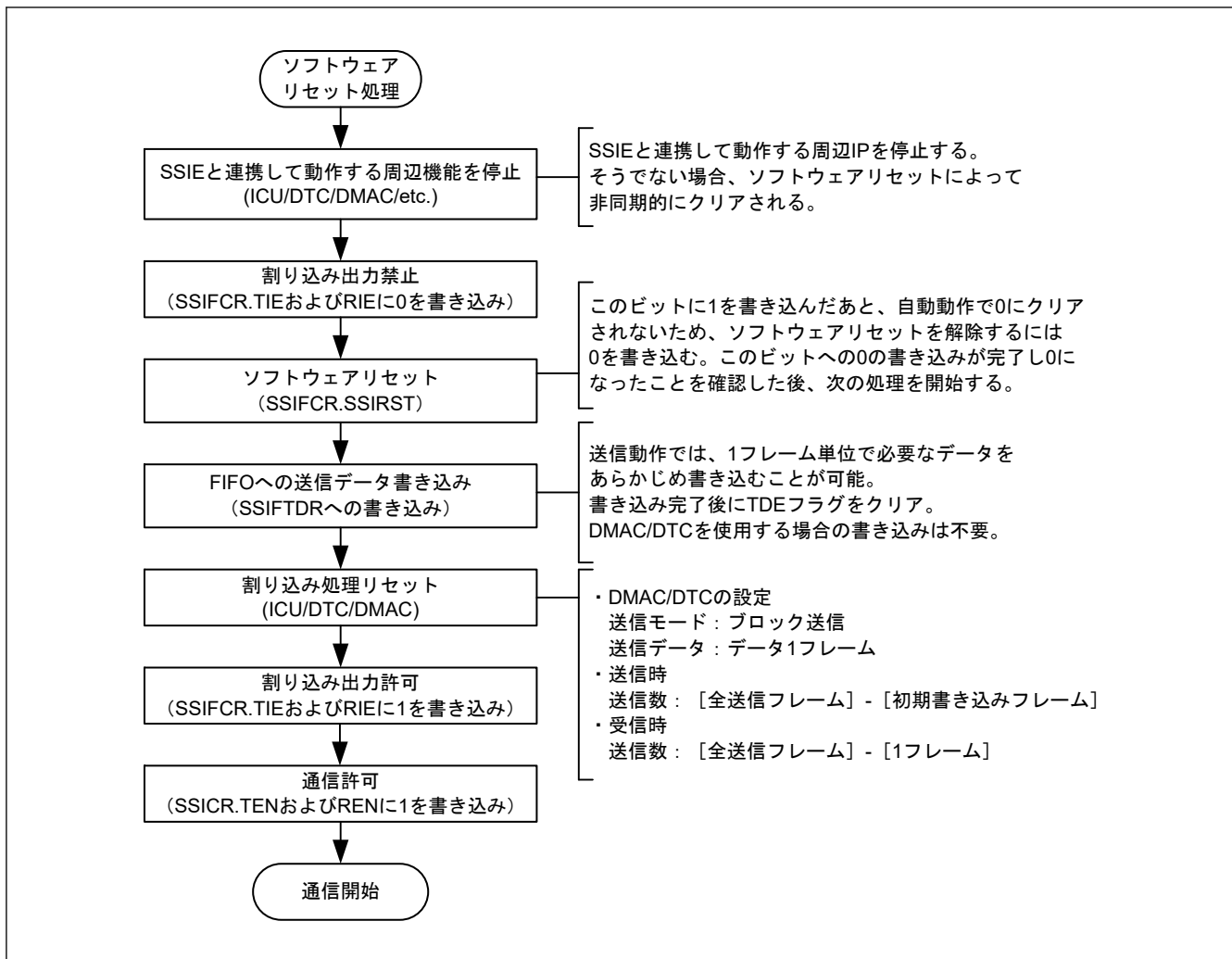
図 39.62 ソフトウェアリセット手順 (CPU 動作手順)
