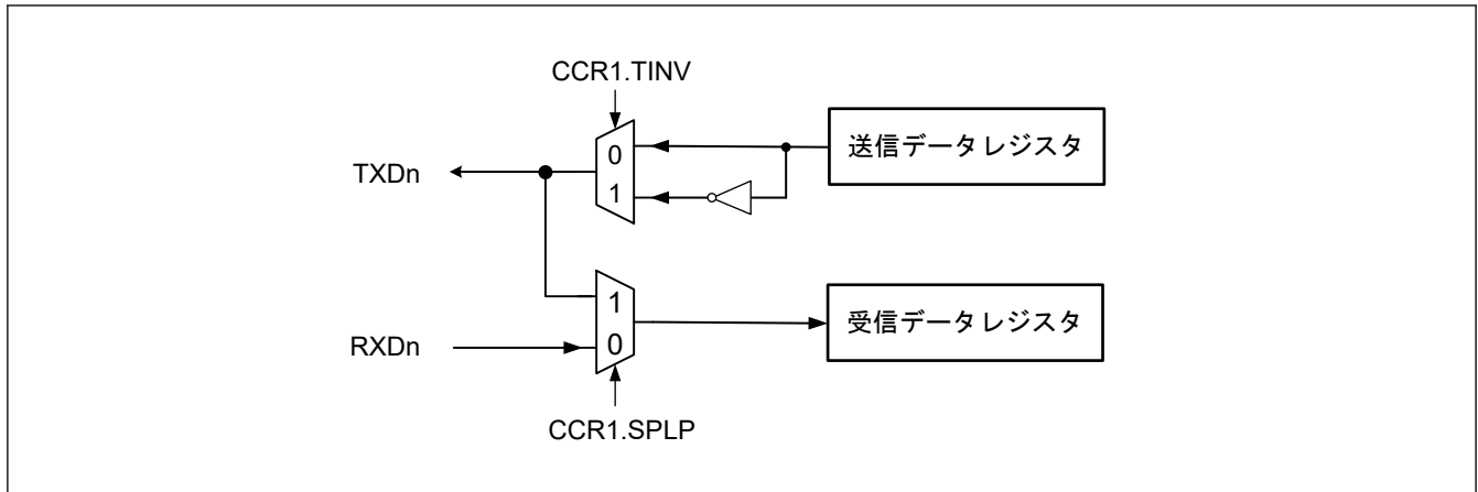
図 31.115 ループバックモードでのシフトレジスタの入出力構成イメージ
