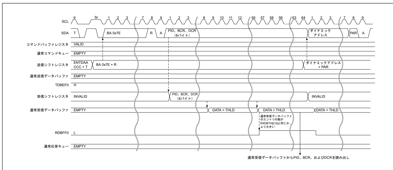
図 33.13 ダイナミックアドレス配置手順 (ENTDAA CCC) タイミング (2/3)
