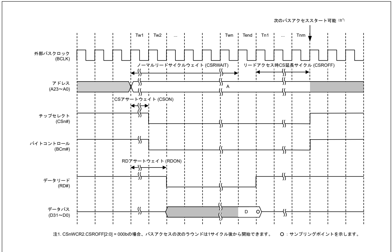
図 14.3 ノーマルリードアクセスのバスタイミング (n = 0~7, m = 0~3)
