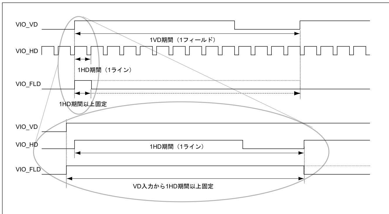
図 53.4 1 フィールドのタイミング
