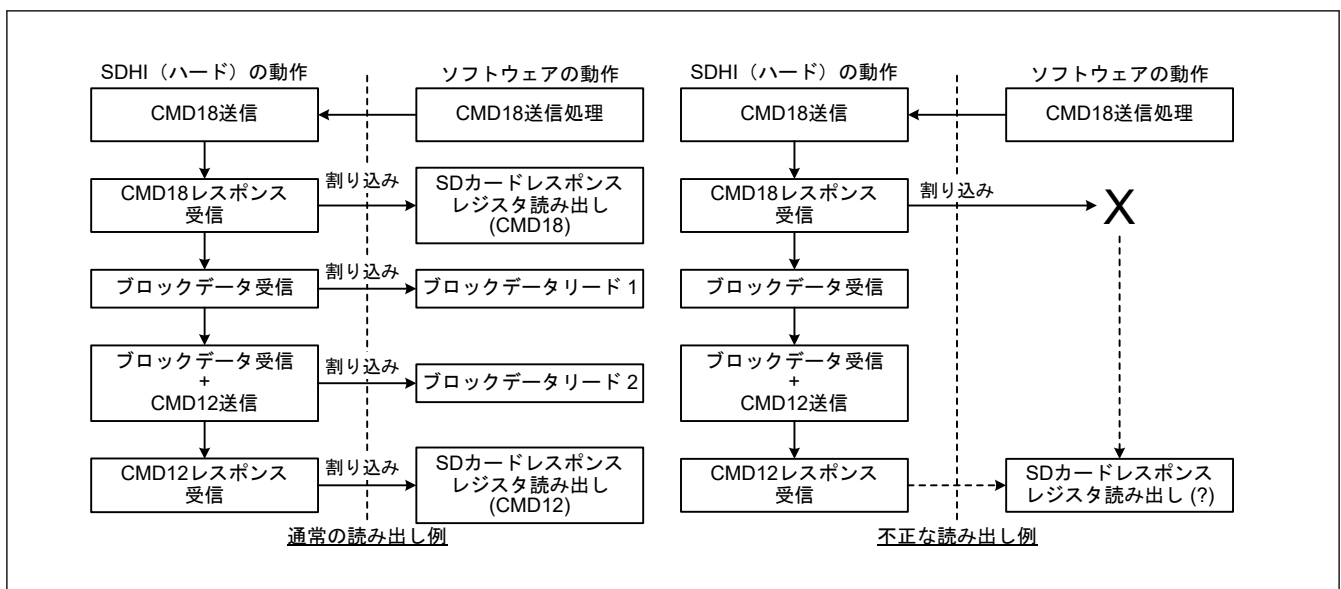
図 40.25 マルチブロックリード動作のフローチャート (2 ブロック)
