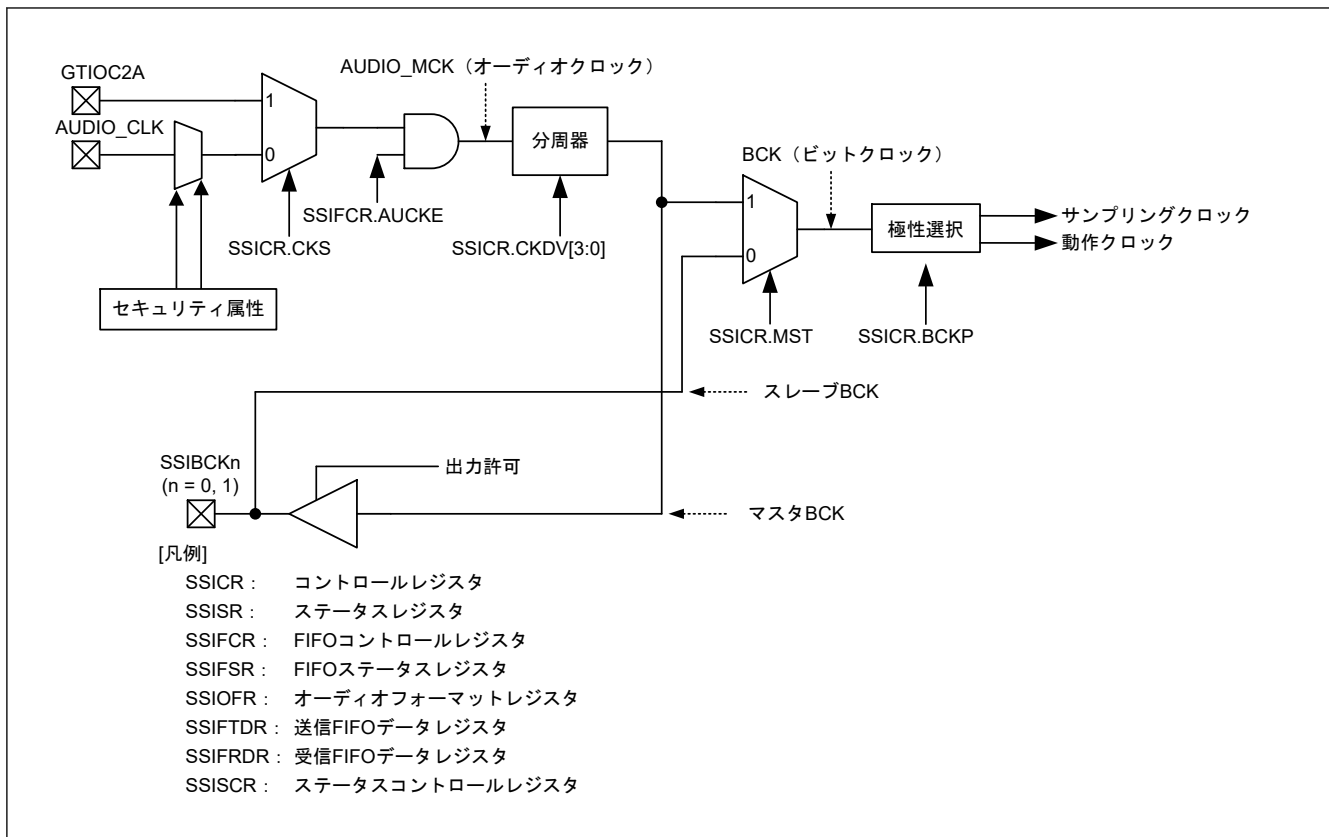
図 39.4 SSIE クロック構成
