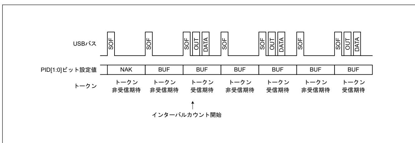
図 30.15 IITV[2:0] ≠ 0 の場合のフレームとトークン受信期待の関係
