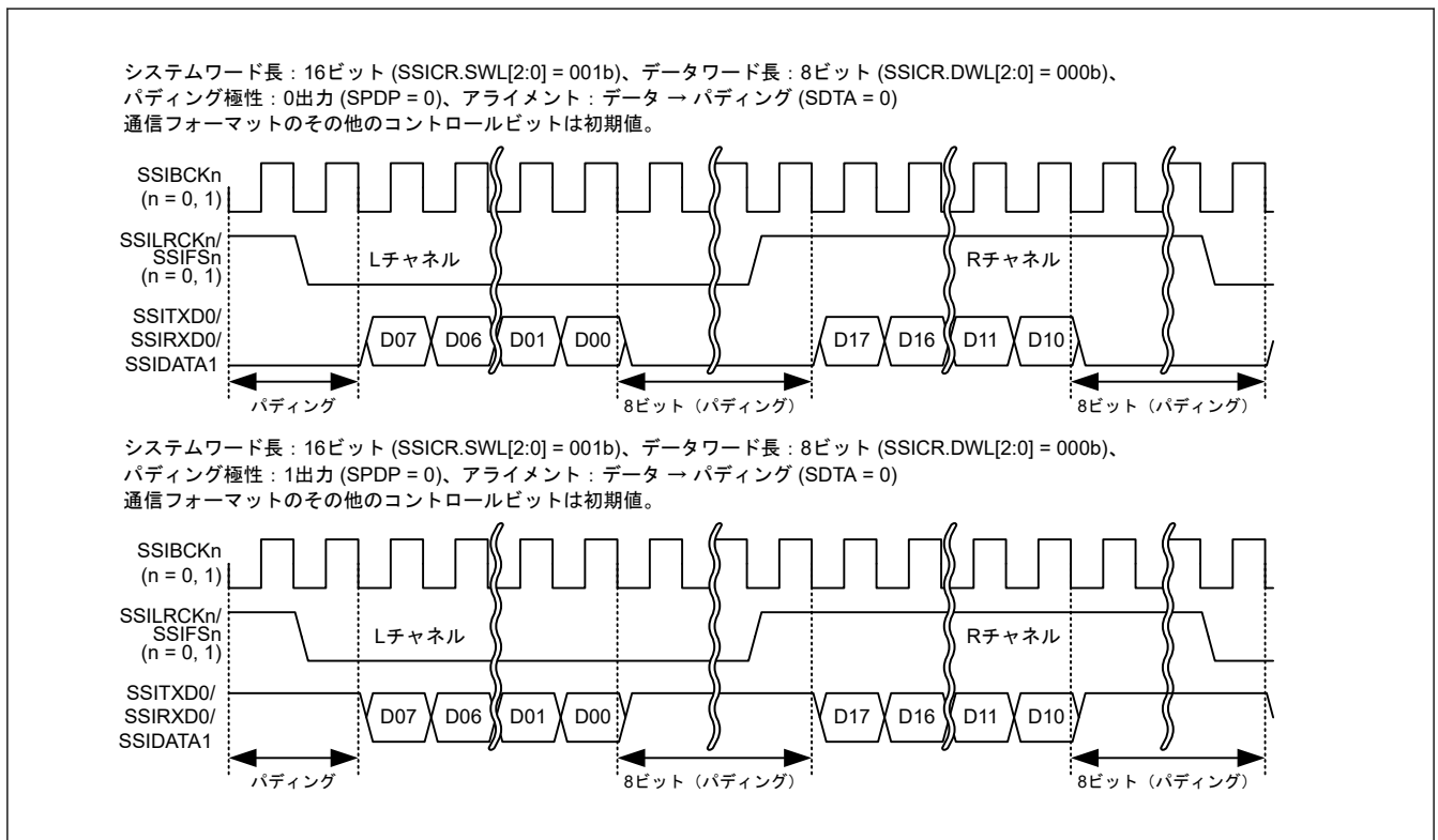
図 39.11 パディングビットの極性
