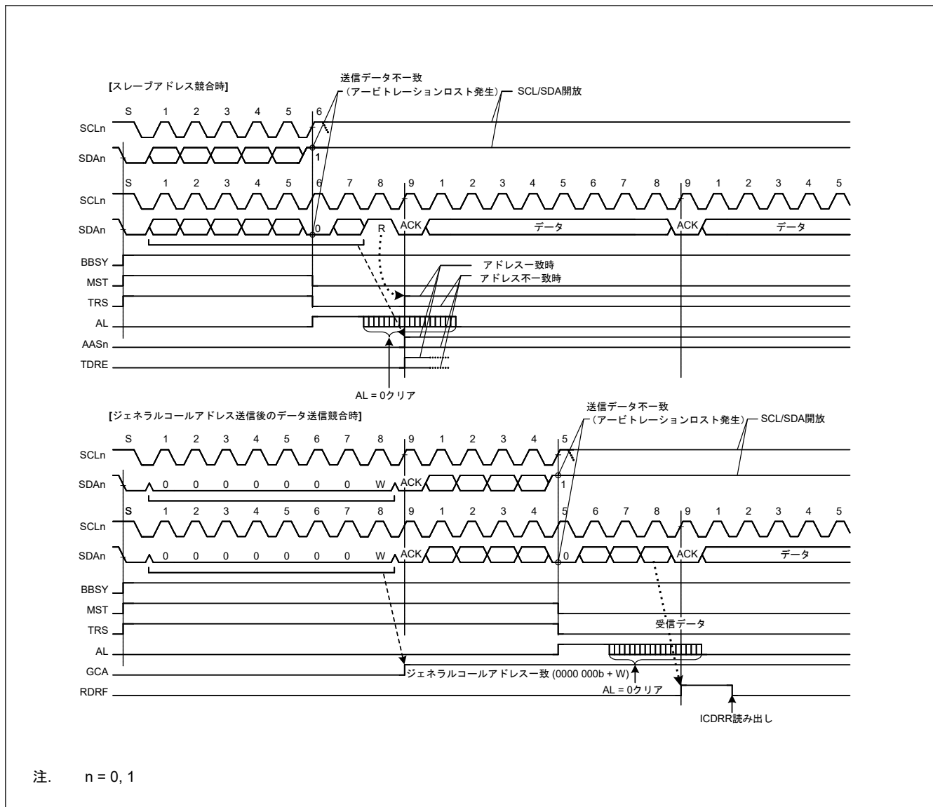
図 32.41 マスタアビトラージョンロスト検出動作例 (MALE = 1 の場合)
