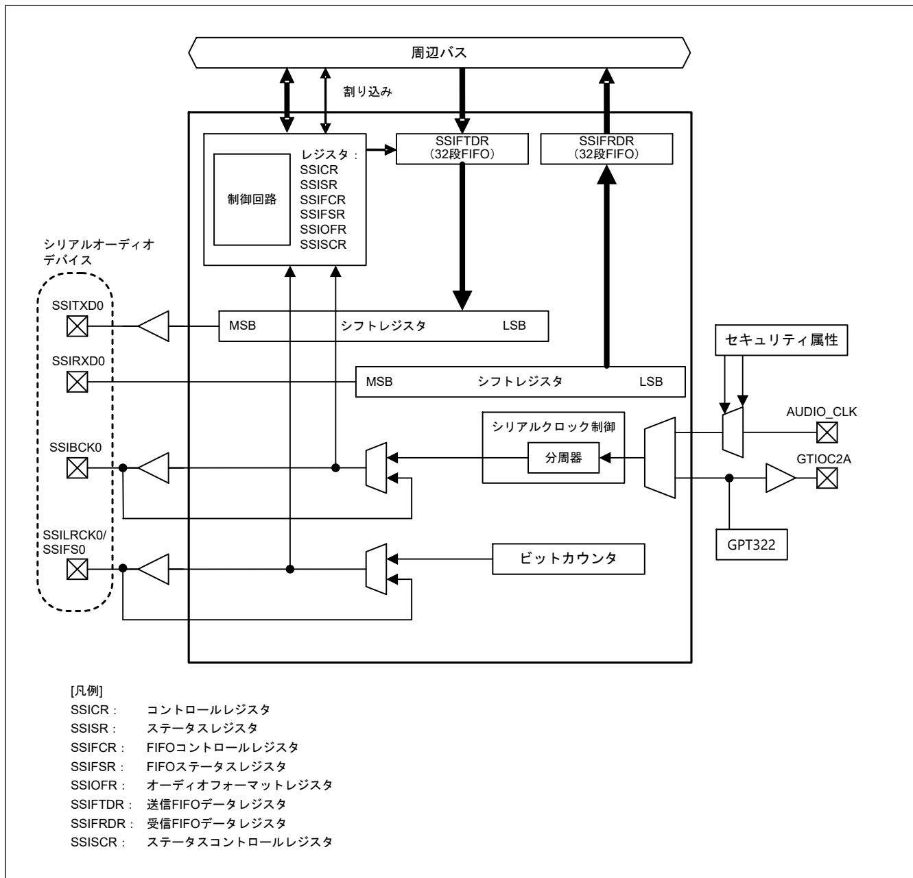
図 39.2 SSIE ブロック図 (SSIE0)
