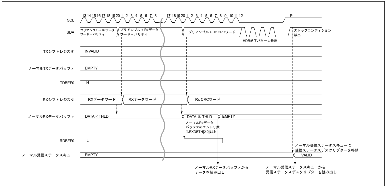
図 33.55 HDR データ書き込み転送 (HDR-DDR) タイミング (3/3)
