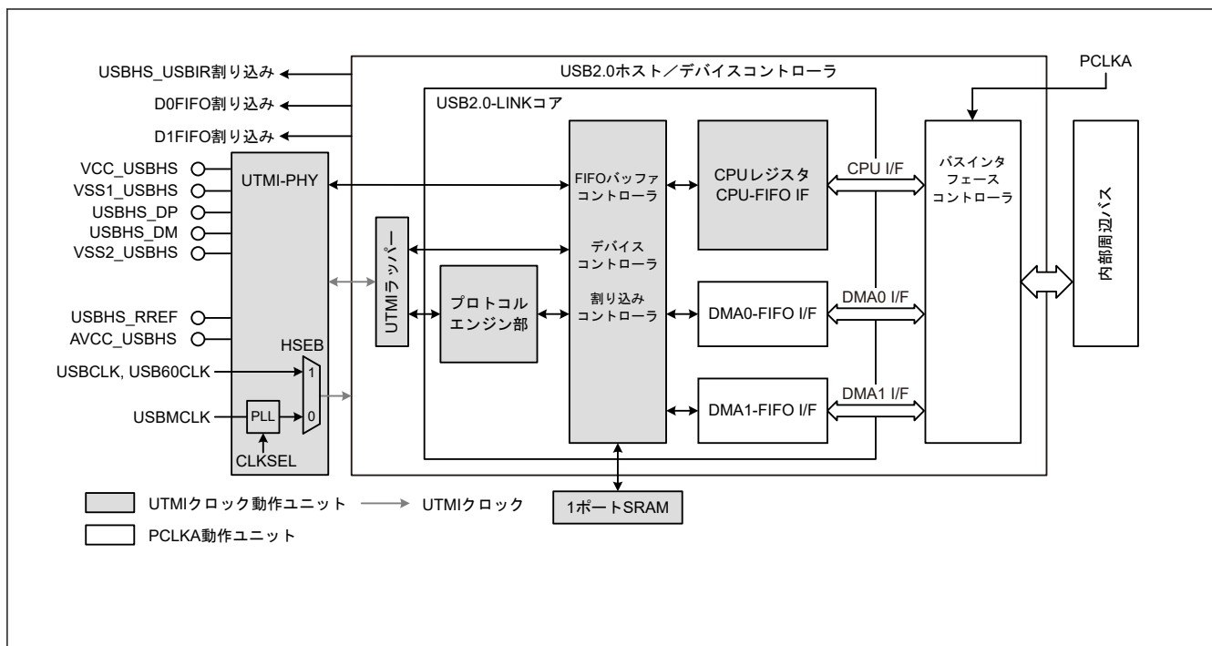
図 30.1 USBHS ブロック図
