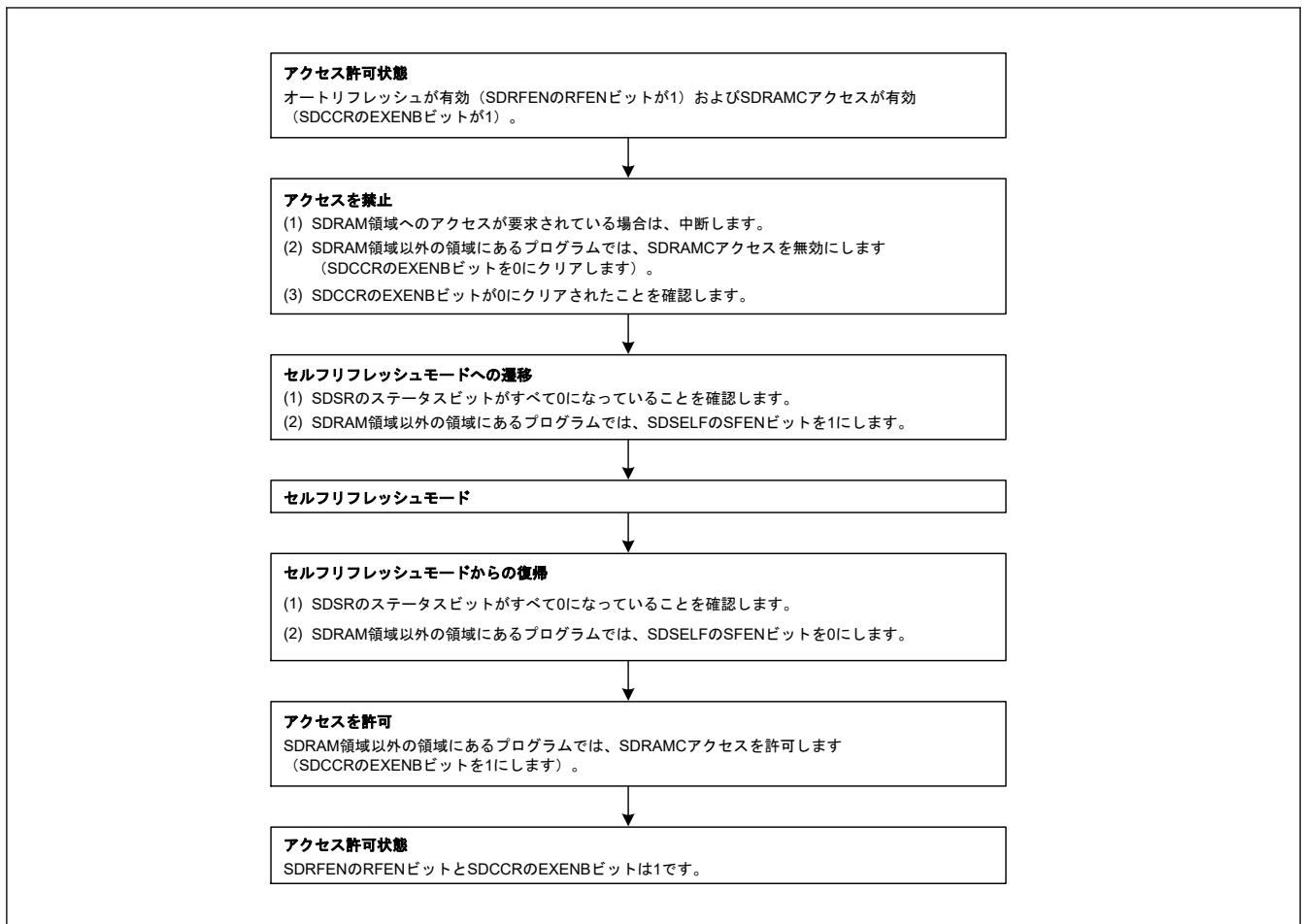
図 14.50 セルフリフレッシュモード遷移／復帰手順
