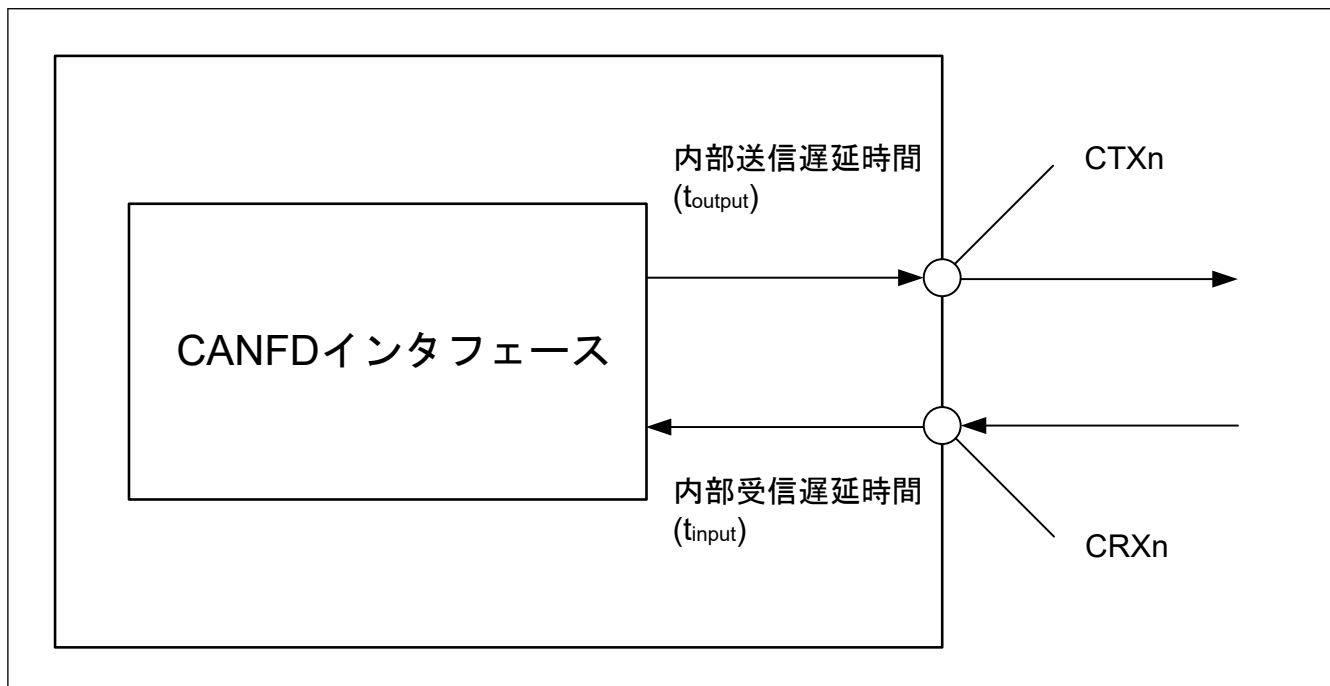
図 55.103 CANFD インタフェース条件
