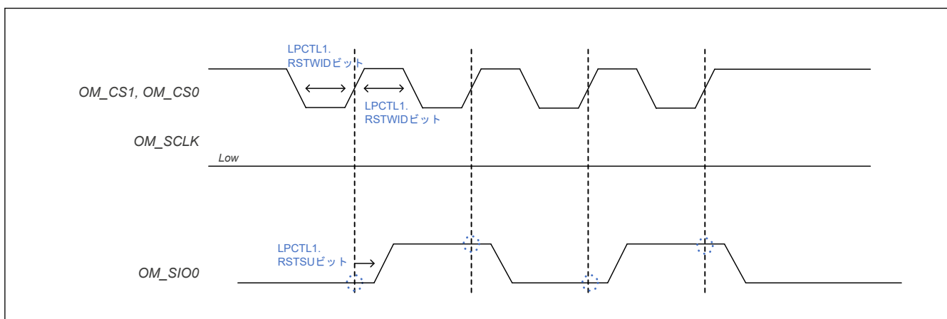
図 37.20 リセットパターン
