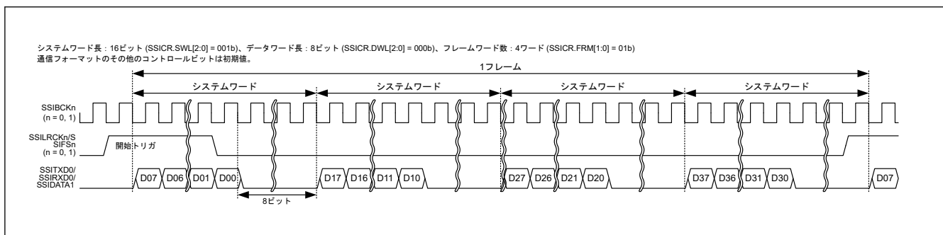
図 39.42 TDM フォーマット (パディングあり、システムワード長 > データワード長)
