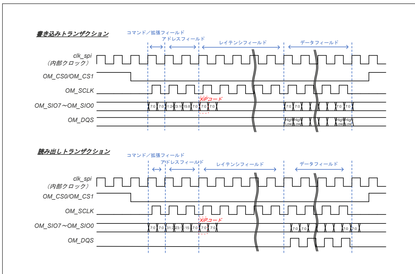
図 37.6 8D-8D-8D プロファイル 1.0 のタイミングチャート
