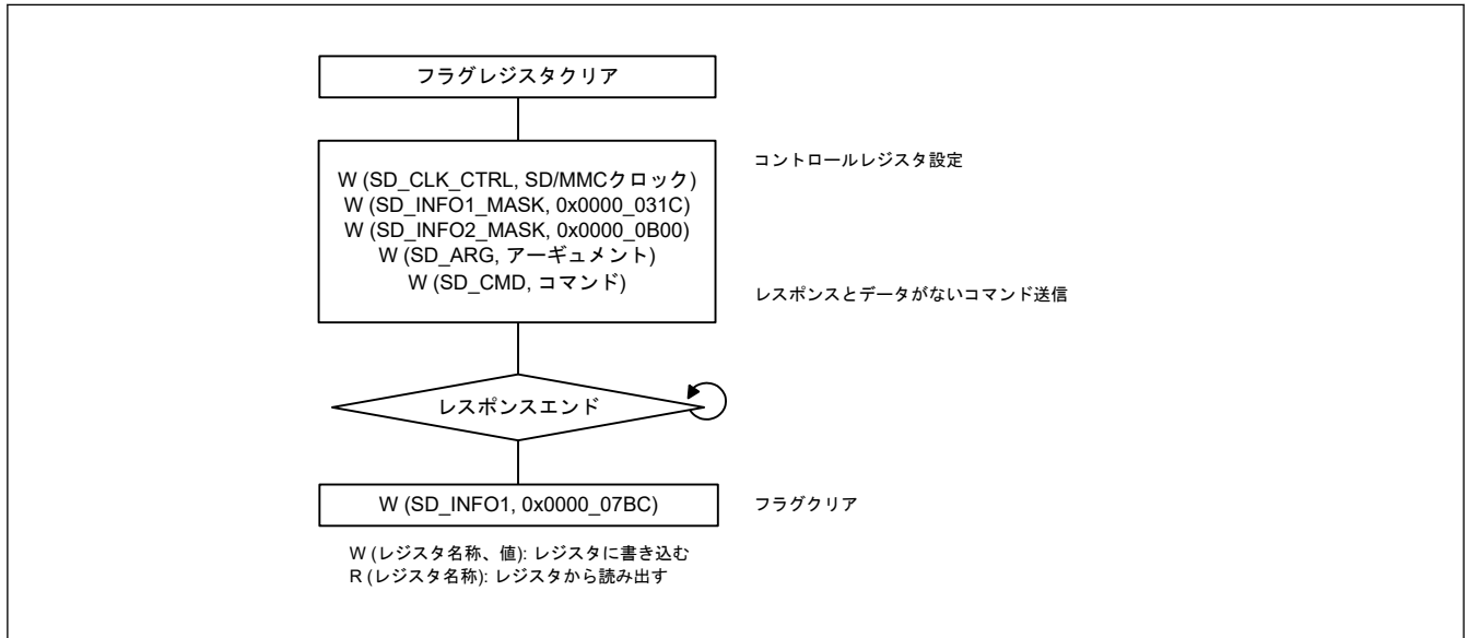
図 40.9 レスポンスまたはデータがないコマンドのフロー例
