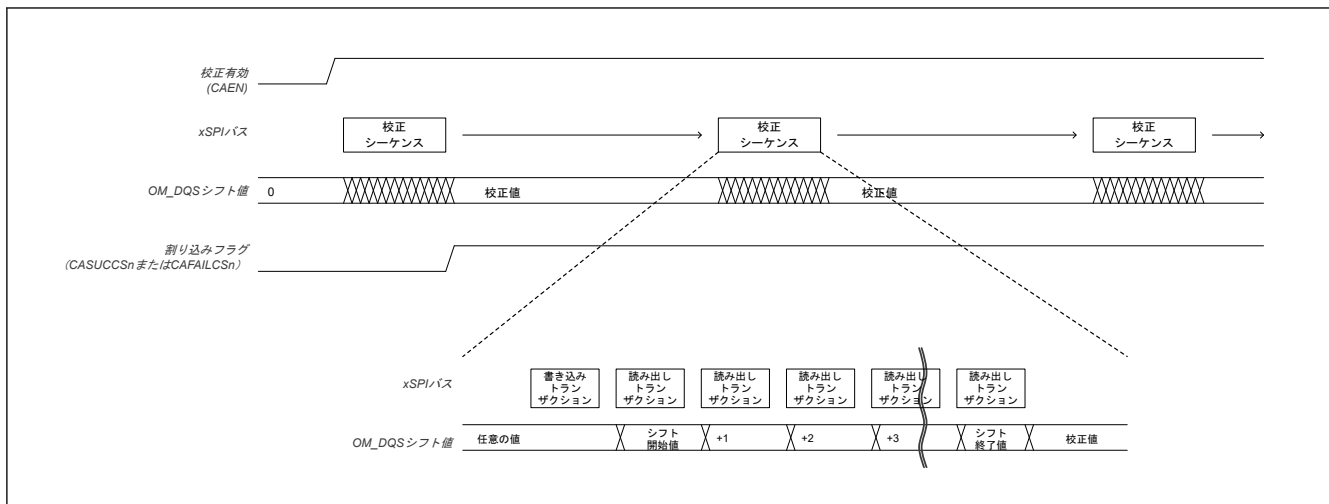
図 37.11 自動校正
