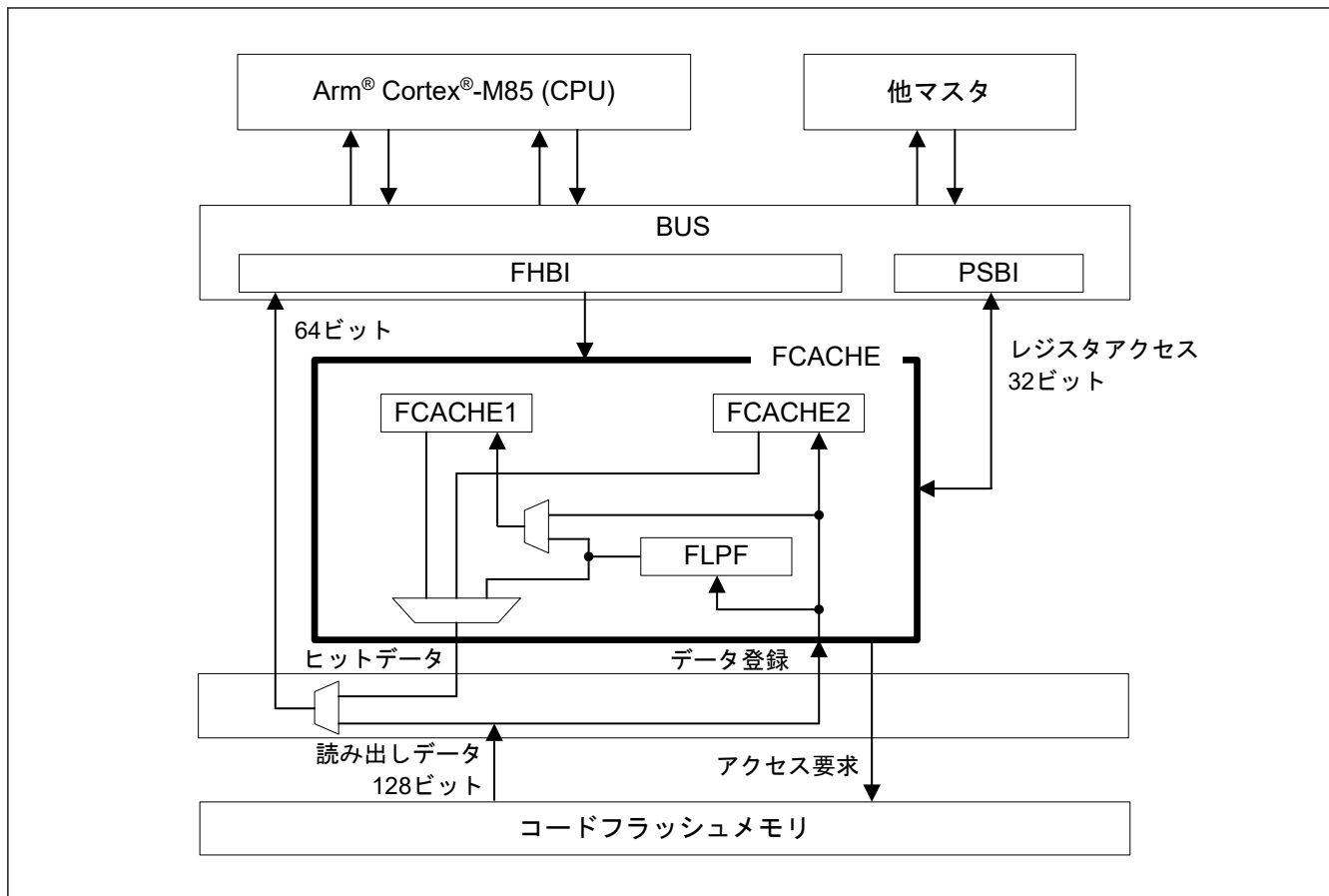
図 52.5 FCACHEのブロック図
