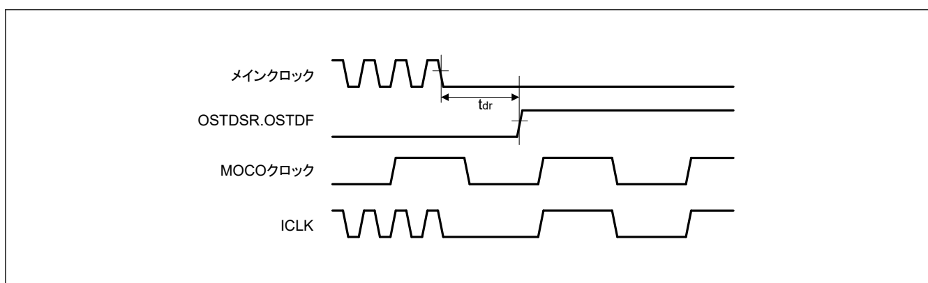
図 55.117 発振停止検出タイミング
