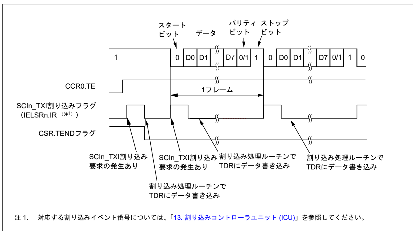
図 31.12 調歩同期式モードにおけるシリアル送信の動作例 (1) (8 ビットデータ/パリティあり/1ストップビット/CTS 機能不使用/送信開始時)
