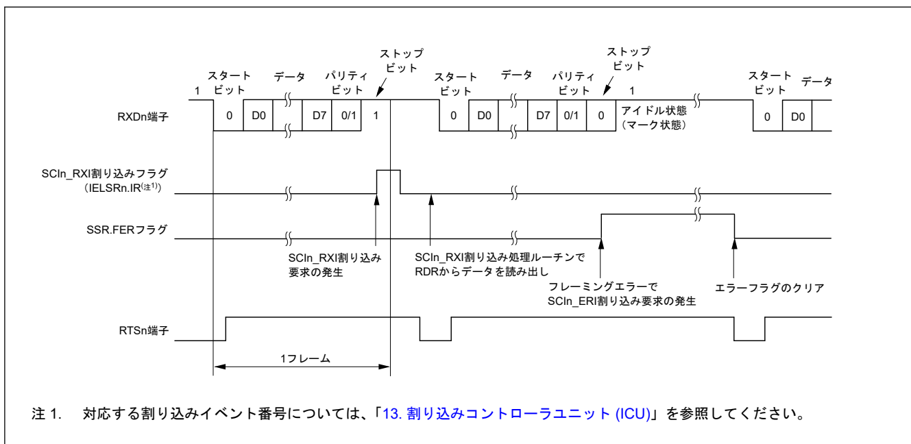
図 31.20 調歩同期式モードにおけるシリアル受信の動作例 (2) (RTS 機能を使用する場合) (8 ビットデータ / パリティあり / 1 ストップビットの場合)
