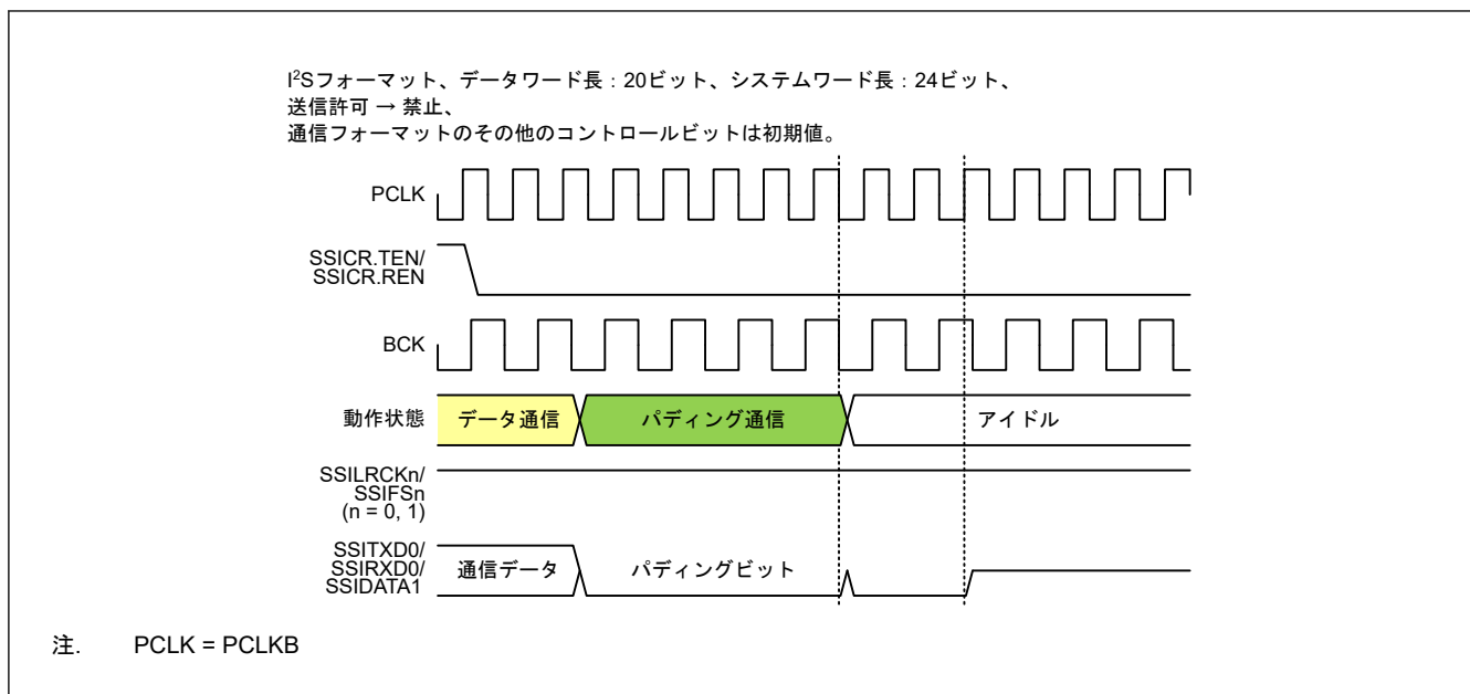
図 39.51 パディング通信からの停止
