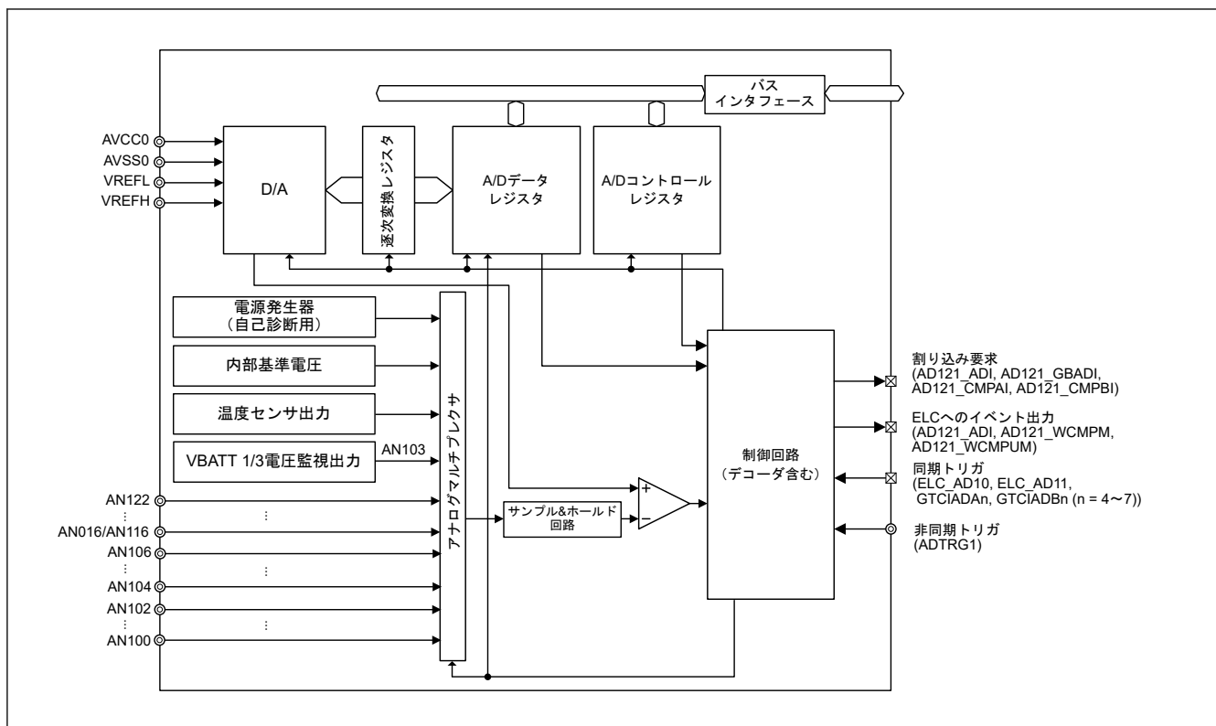
図 45.2 ADC12 のブロック図 (ユニット 1)
