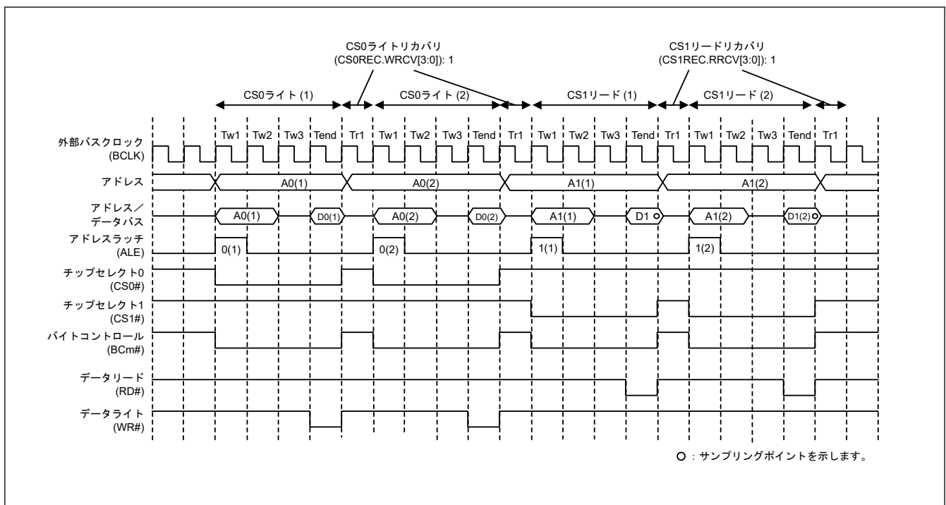
図 14.34 バスアクセスが分割された場合のリカバリサイクルの動作例 (アドレス/データマルチプレクス I/O インタフェースの場合) (m = 0, 1)
