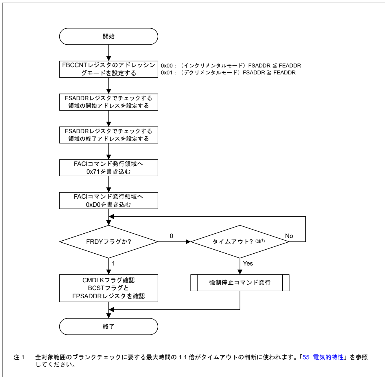
図 52.24 ブランクチェックコマンドの使用フロー
