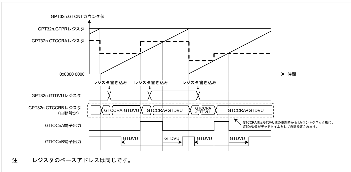
図 21.26 デッドタイム自動設定機能の動作例 (のこぎり波ワンショットパルスモード、アップカウント、アクティブ High の場合)
