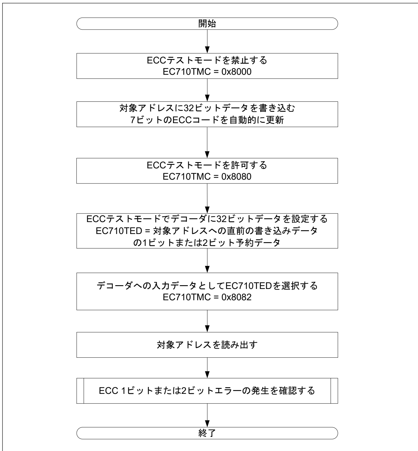
図 35.2 ECC デコーダのテスト手順
