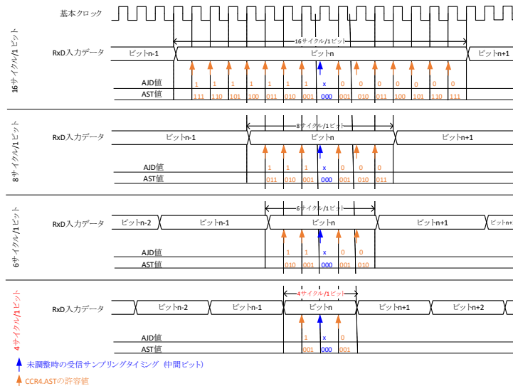
図 31.29 受信サンプリングタイミングの調整動作の概要 (内部クロックを使用した調歩同期式モード)
