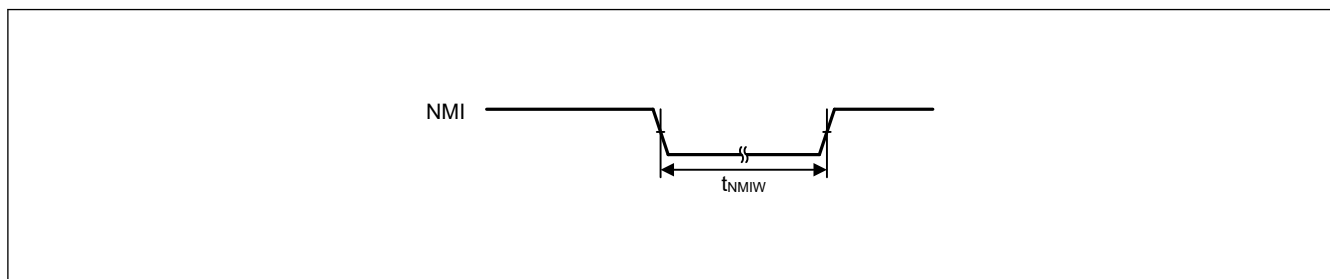
図 55.26 NMI 割り込み入カタイミング
