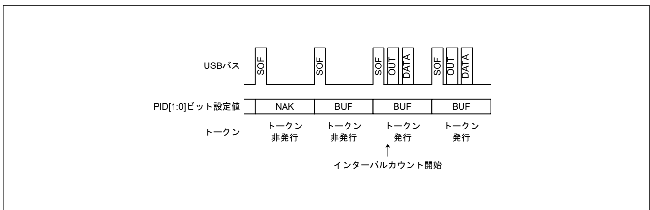
図 30.12 IITV[2:0] = 0 の場合におけるトークン発行の有無
