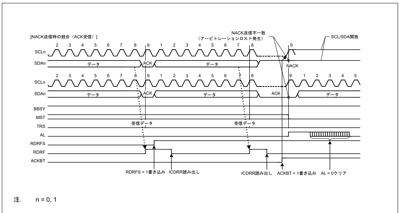
図 32.43 NACK 送信中のアービトレーションロスト検出の動作例 (NALE = 1 の場合)
