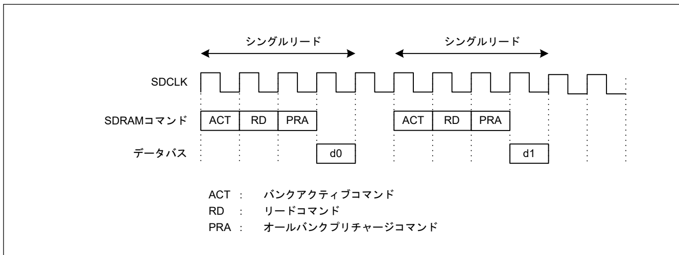
図 14.43 シングルリードのタイミング例 (SDTR.CL[2:0] = 010b : 2 サイクル)
