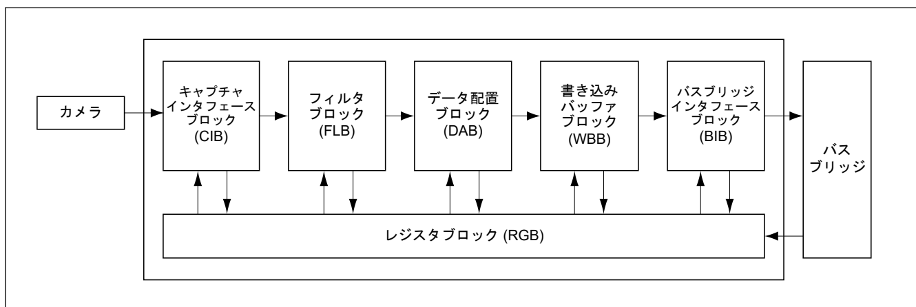
図 53.1 CEU のブロック図
