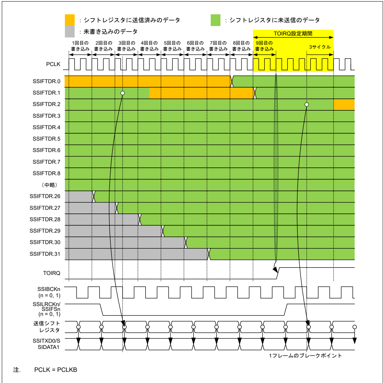
図 39.18 TOIRQ 設定タイミング
