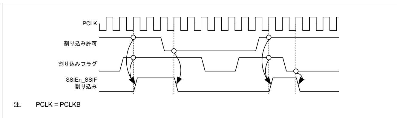
図 39.59 共通割り込み要因のタイミング図 (SSIEn_SSIF)
