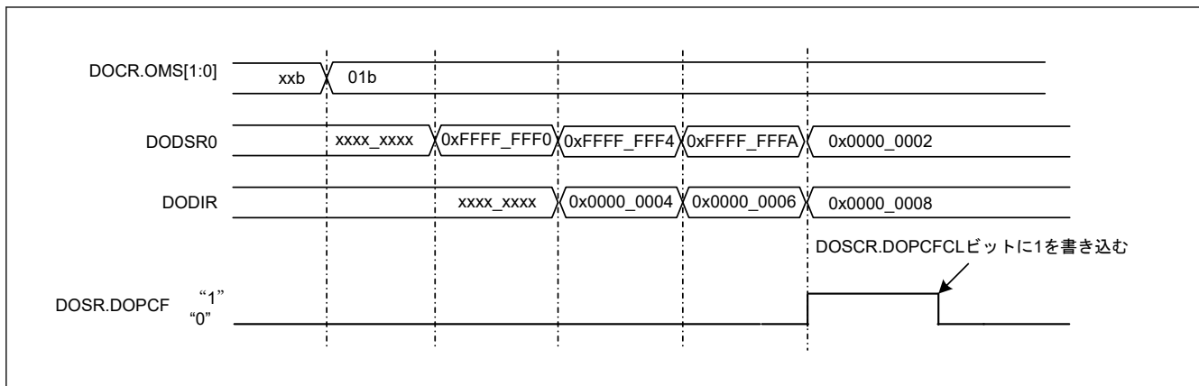
図 49.8 データ加算モードの動作例
