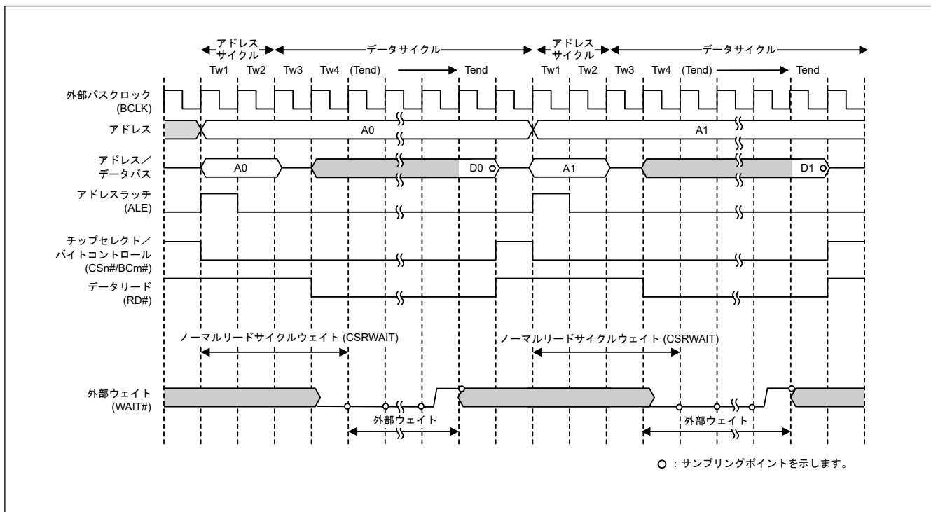
図 14.28 アドレス/データマルチプレクス I/O インタフェース時の外部ウェイト挿入のタイミング例 (n = 0~7, m = 0, 1)
