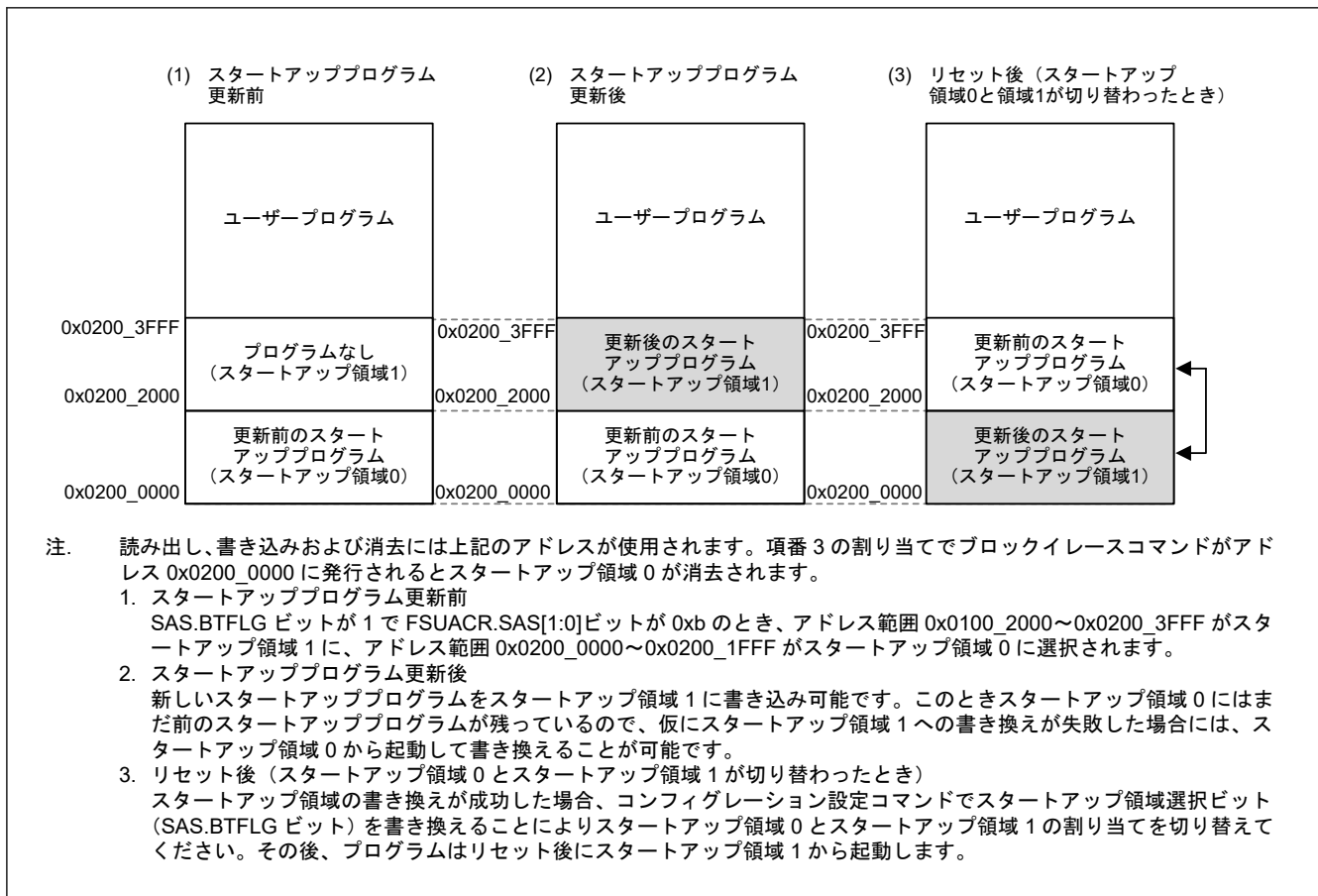
図 52.29 スタートアッププログラムプロテクションの概念 (セキュアエアリアスの場合)
