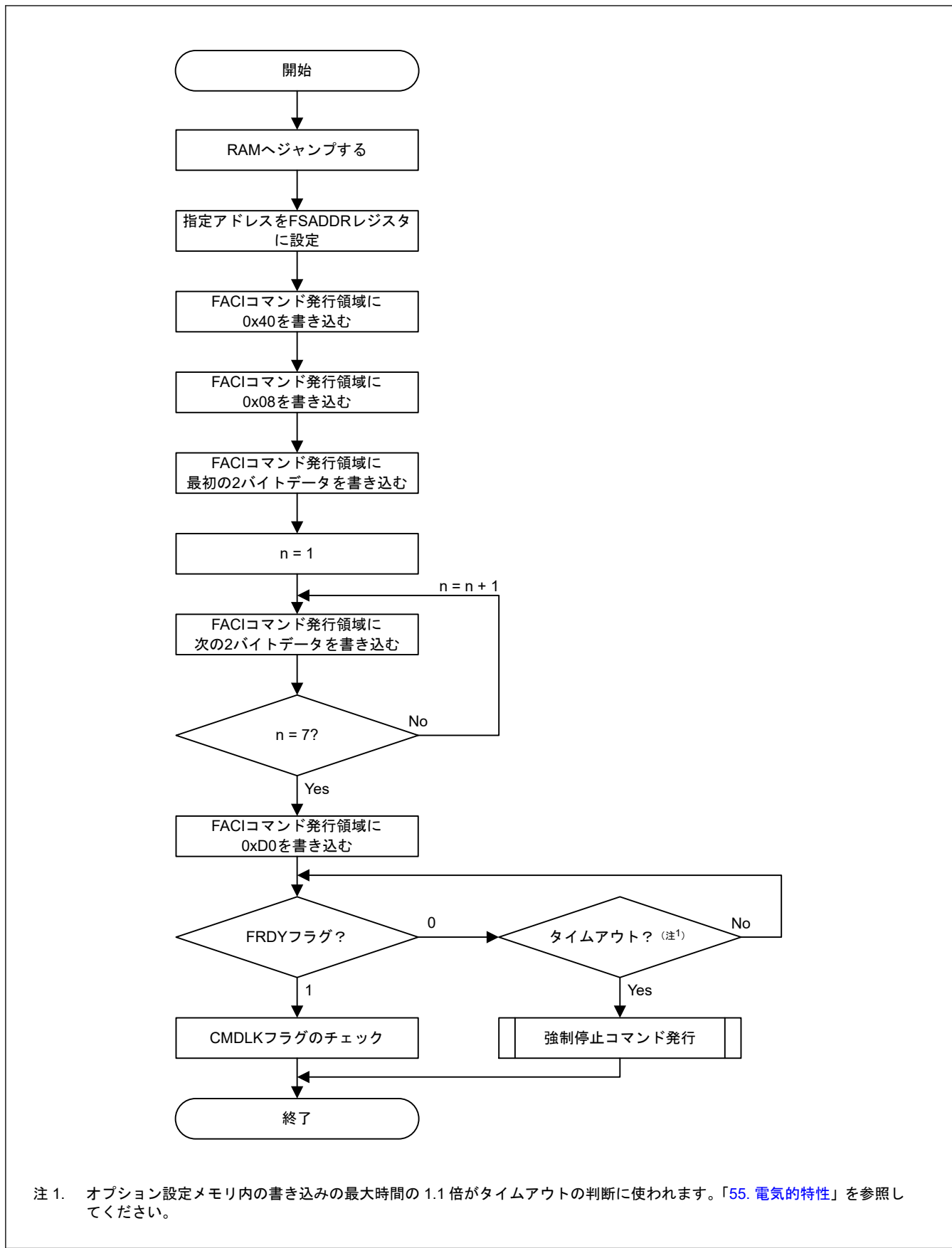
図 52.25 コンフィグレーション設定コマンドの使用フロー
