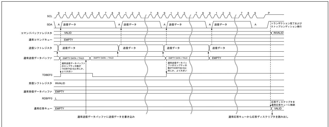
図 33.19 レガシー I 2 C メッセージデータ書き込みタイミング (2/2)
