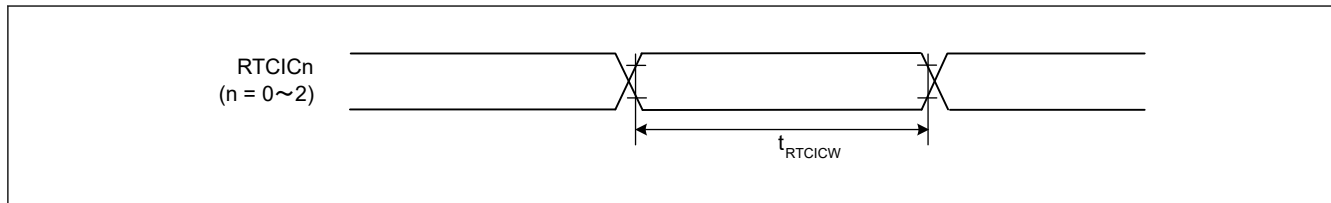
図 55.43 RTCICn 入力タイミング
