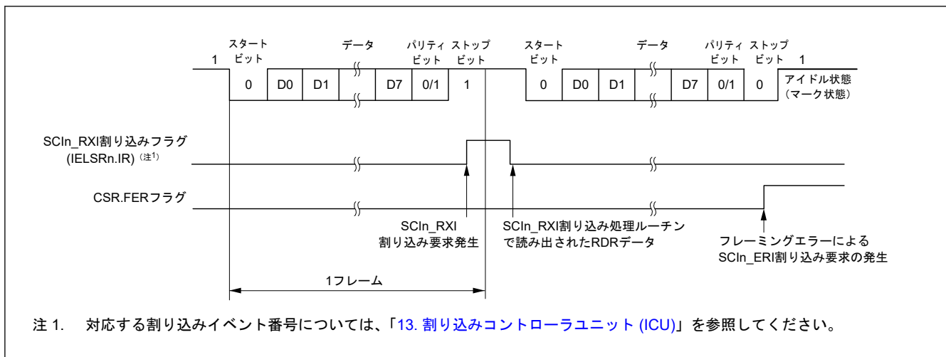
図 31.19 調歩同期式モードにおけるシリアル受信の動作例 (1) (RTS 機能を使用しない場合) (8 ビットデータ / パリティあり / 1 ストップビットの場合)
