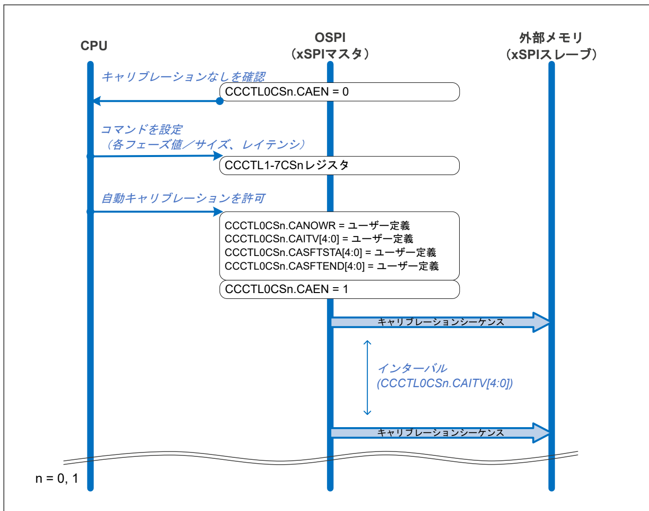
図 37.24 自動校正のフロー
