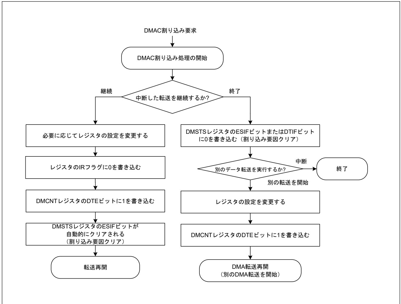
図 16.24 DMAC 割り込み処理ルーチンで DMA 転送を再開/終了する手順
