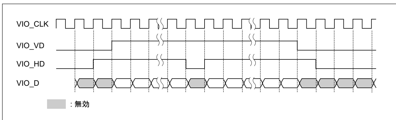
図 53.13 データイネーブル取り込みタイミング (VD が High の期間外に HD がアサート (High))
