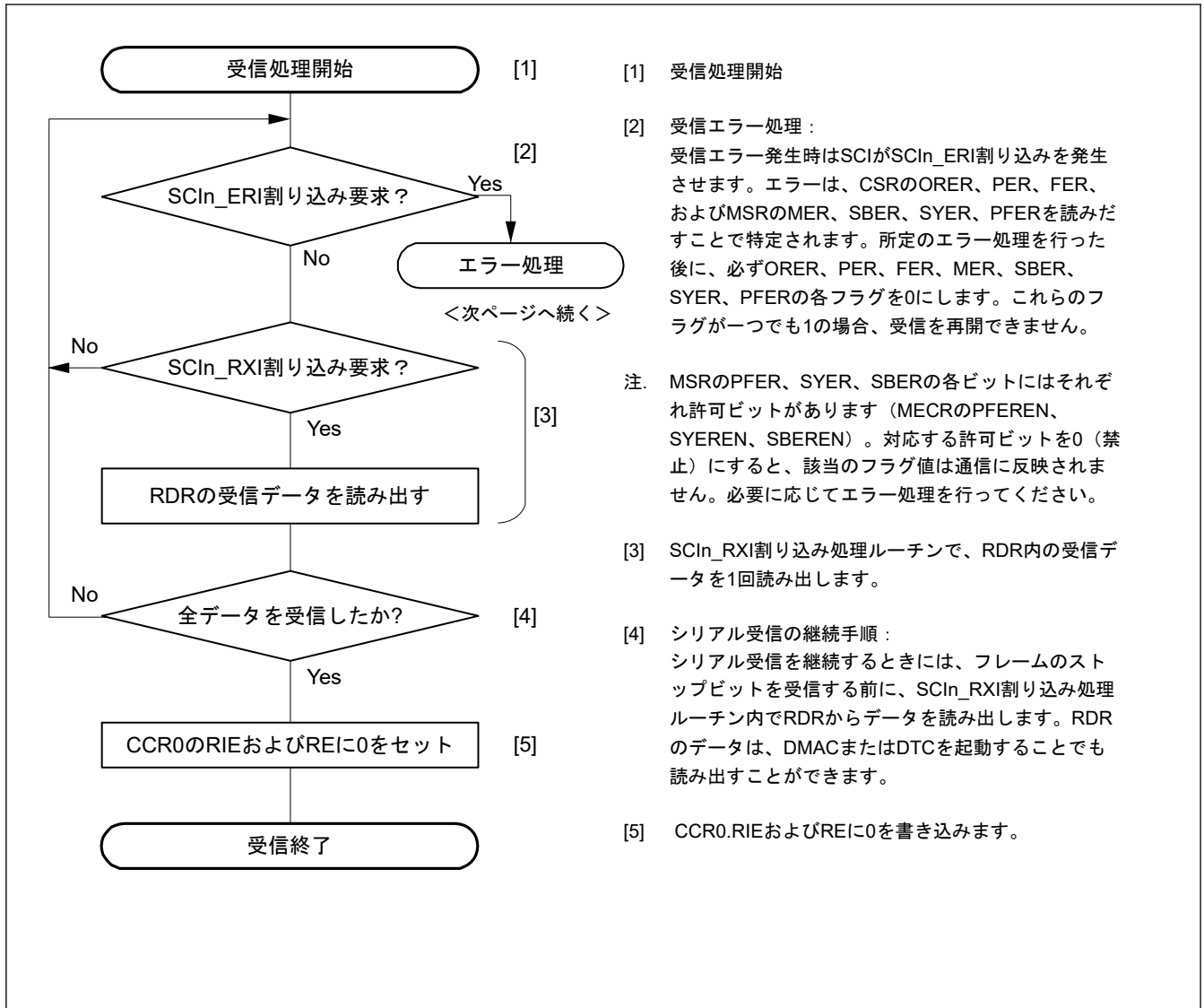
図 31.57 マンチェスタモードにおけるシリアルデータ受信フローチャートの例（正常受信）
