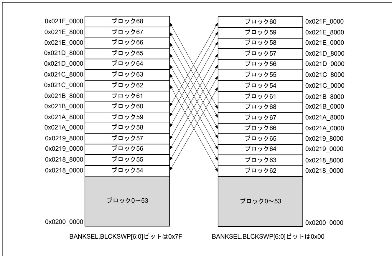
図 52.35 ブロックスワップ選択例（セキュアエイリアスの場合）（2 MB のコードフラッシュメモリを持つ製品の場合）
