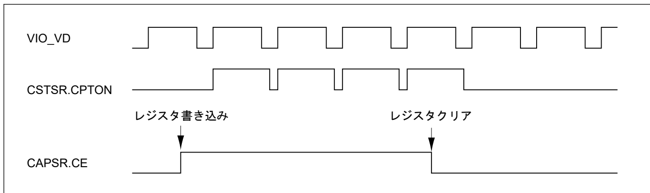
図 53.8 連続フレームキャプチャ
