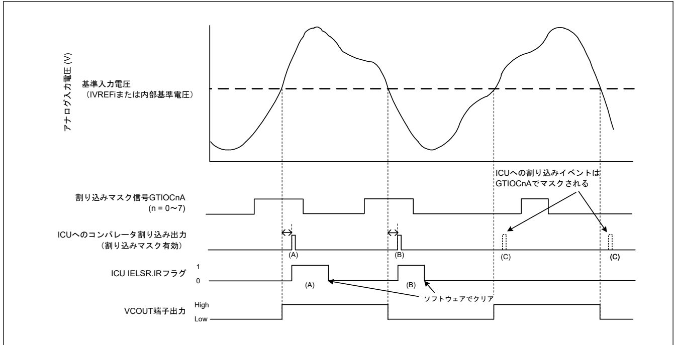
図 48.3 ACMPHS の動作例 (割り込みマスク機能有効)
