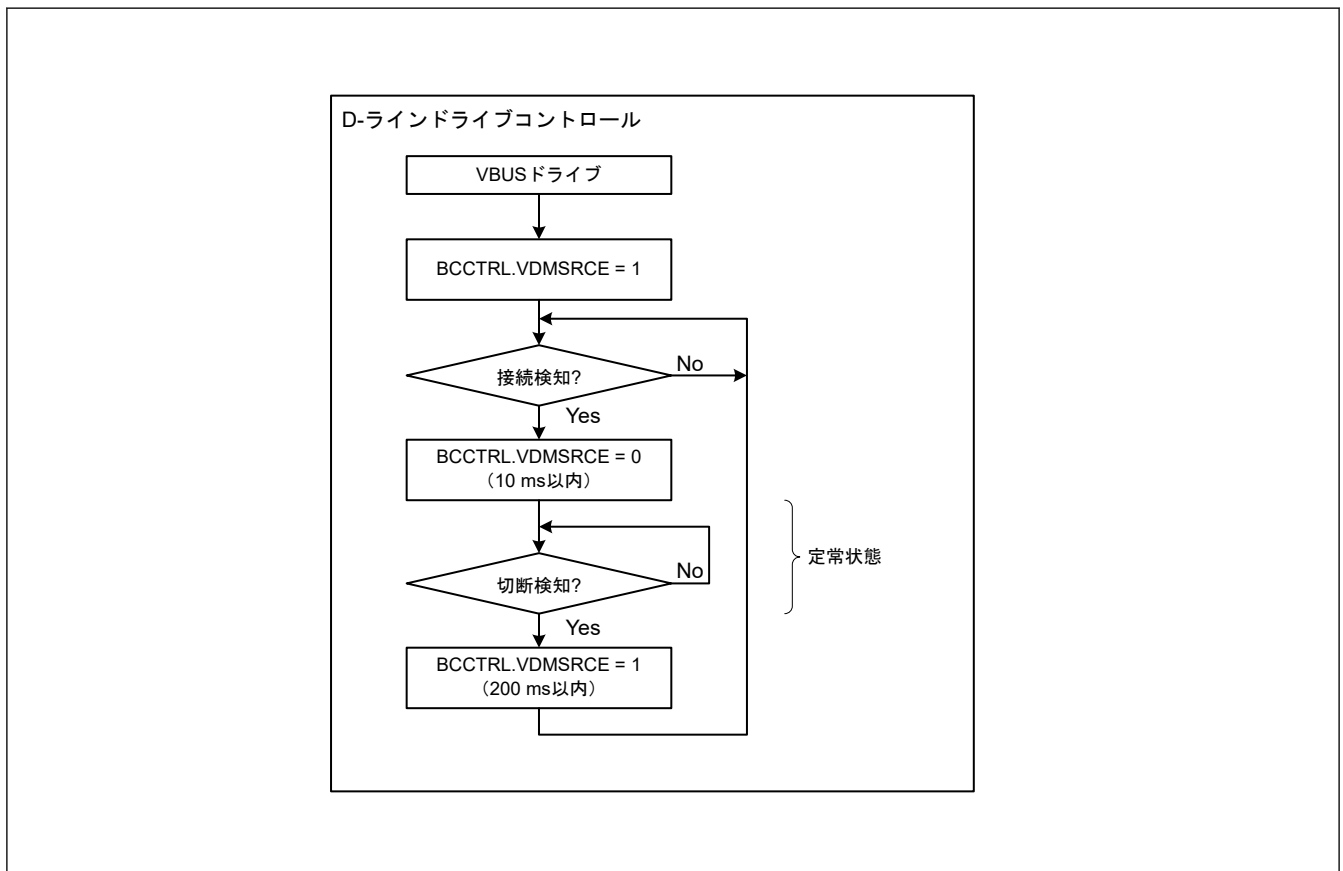
図 30.20 ハードウェアに Portable Device 検出機能未搭載または未使用時の Charging Downstream ポート処理フロー
