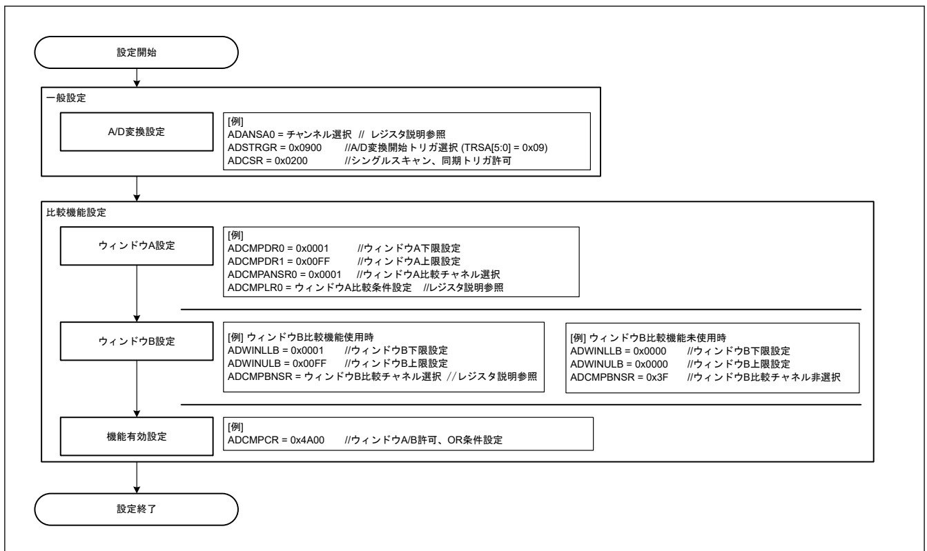
図 45.33 コンペア機能のイベント出力使用時の設定例
