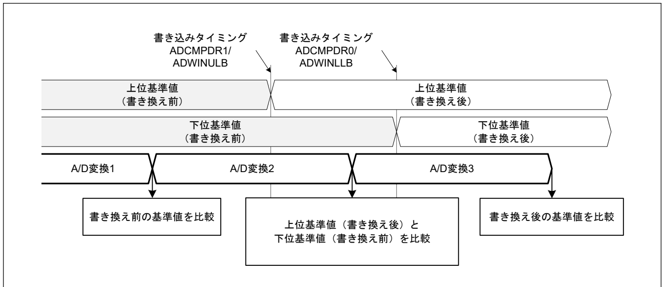
図 45.6 書き換え前後の上側基準値と下側基準値の比較
