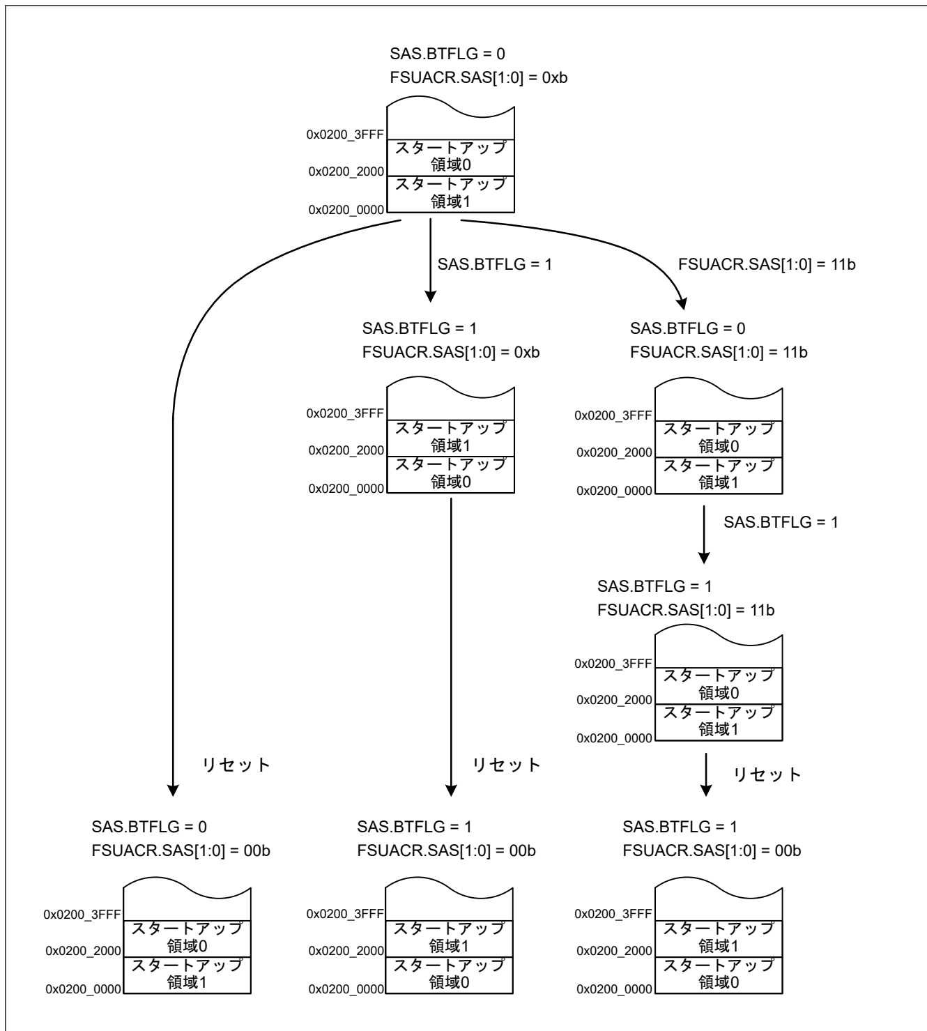
図 52.31 スタートアッププログラム保護設定の遷移例 2 (セキュアエリアの場合)
