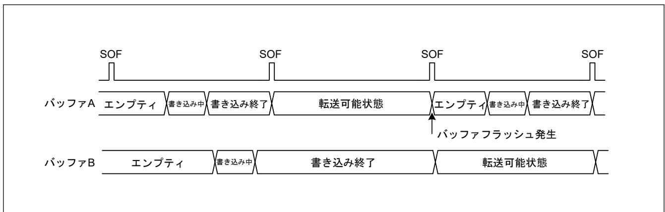
図 30.17 バッファフラッシュ動作例
