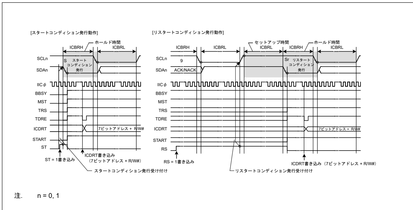
図 32.45 スタートコンディション/リスタートコンディション発行動作タイミング (ST、RS ビット)
