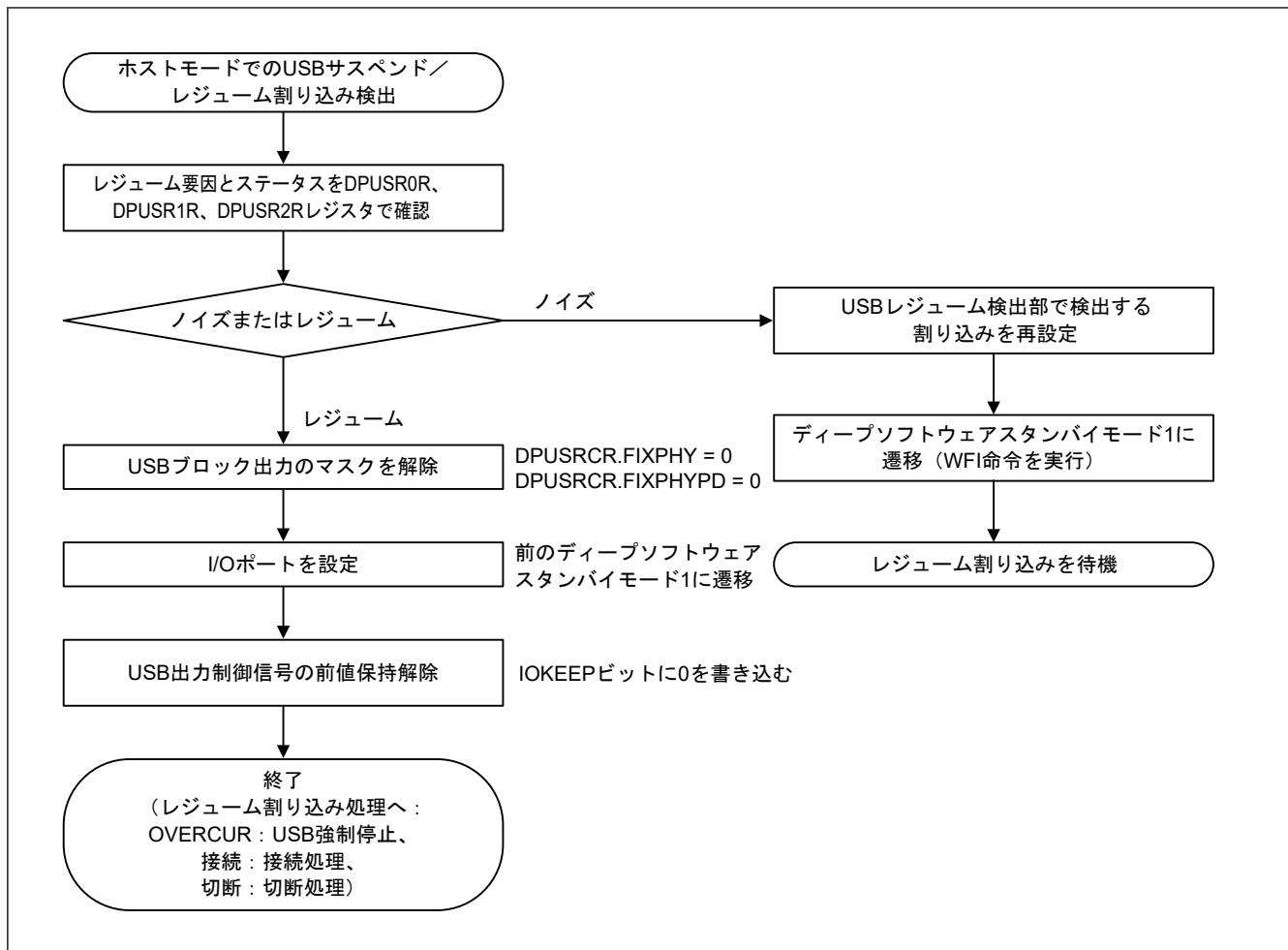
図 30.23 ホストコントローラとしてディープソフトウェアスタンバイモード1を解除する場合のUSBHS 設定フロー (1)
