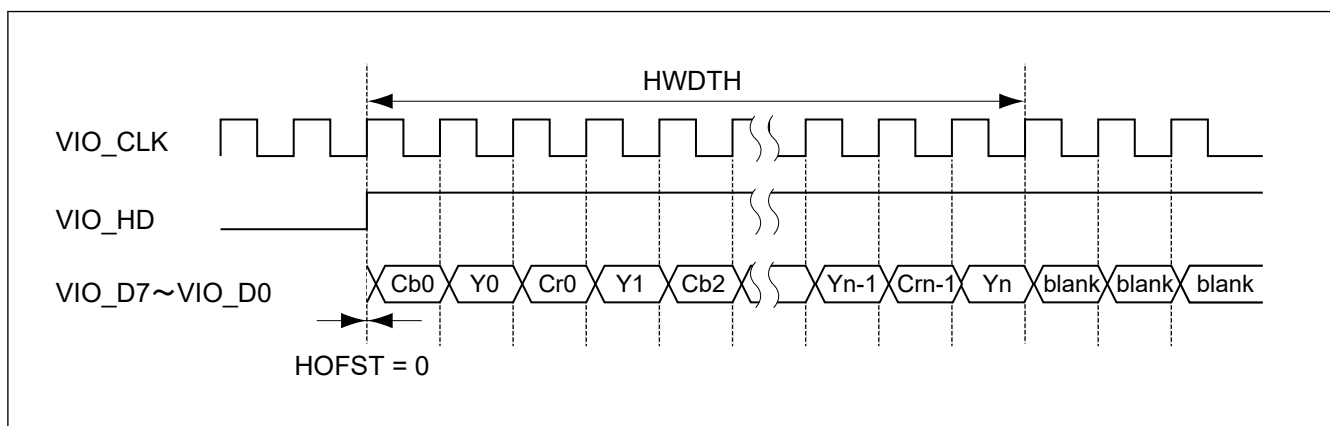
図 53.22 水平キャプチャタイミング (画像キャプチャ 8 ビットインタフェース)
