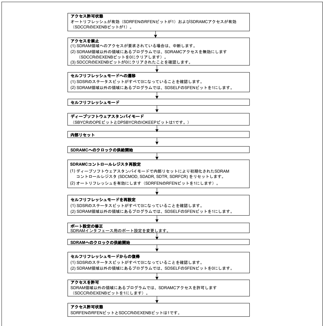
図 14.51 ディープソフトウェアスタンバイモードでのセルフリフレッシュモード遷移／復帰手順
