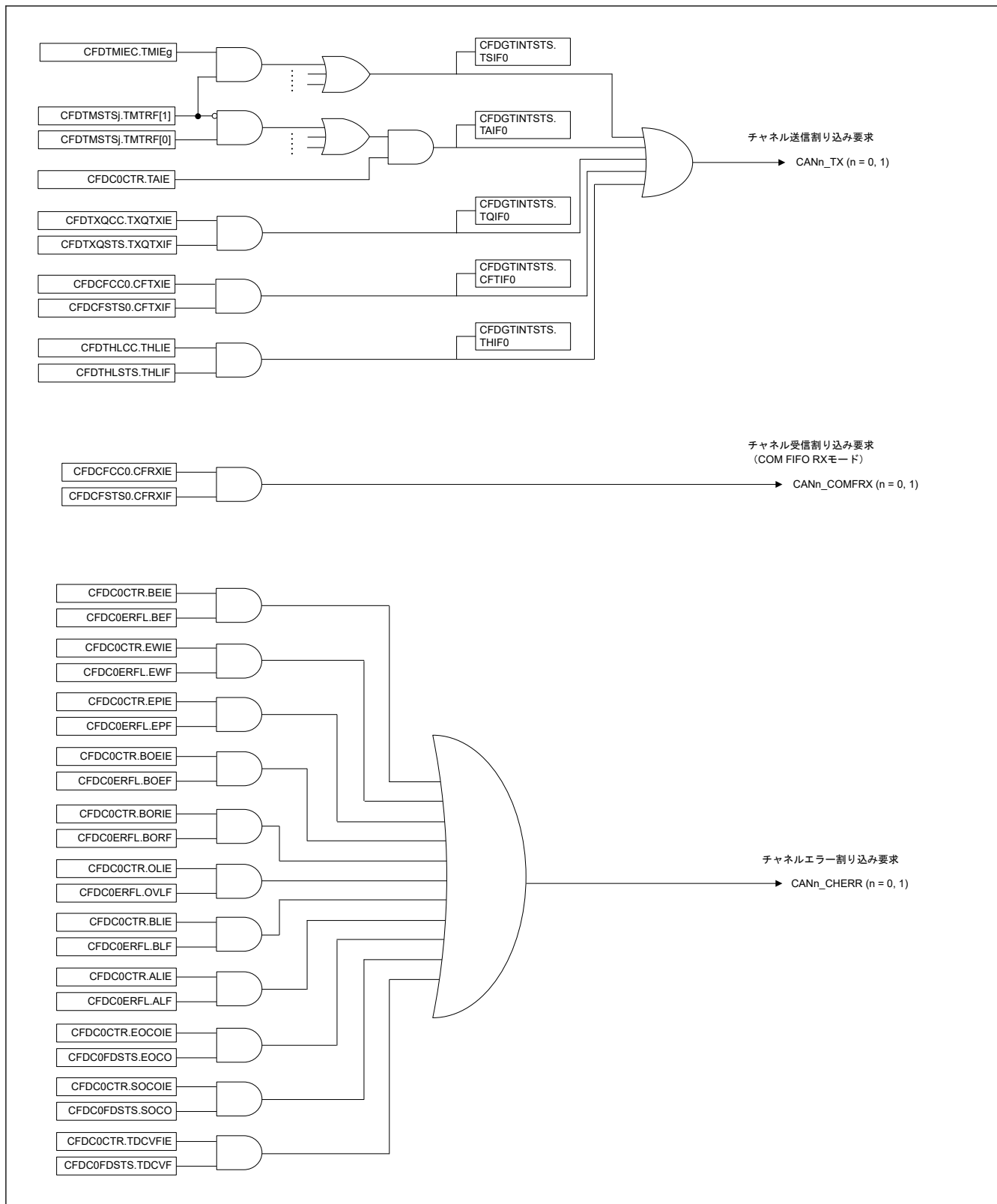
図 34.31 チャネル割り込みのブロック図
