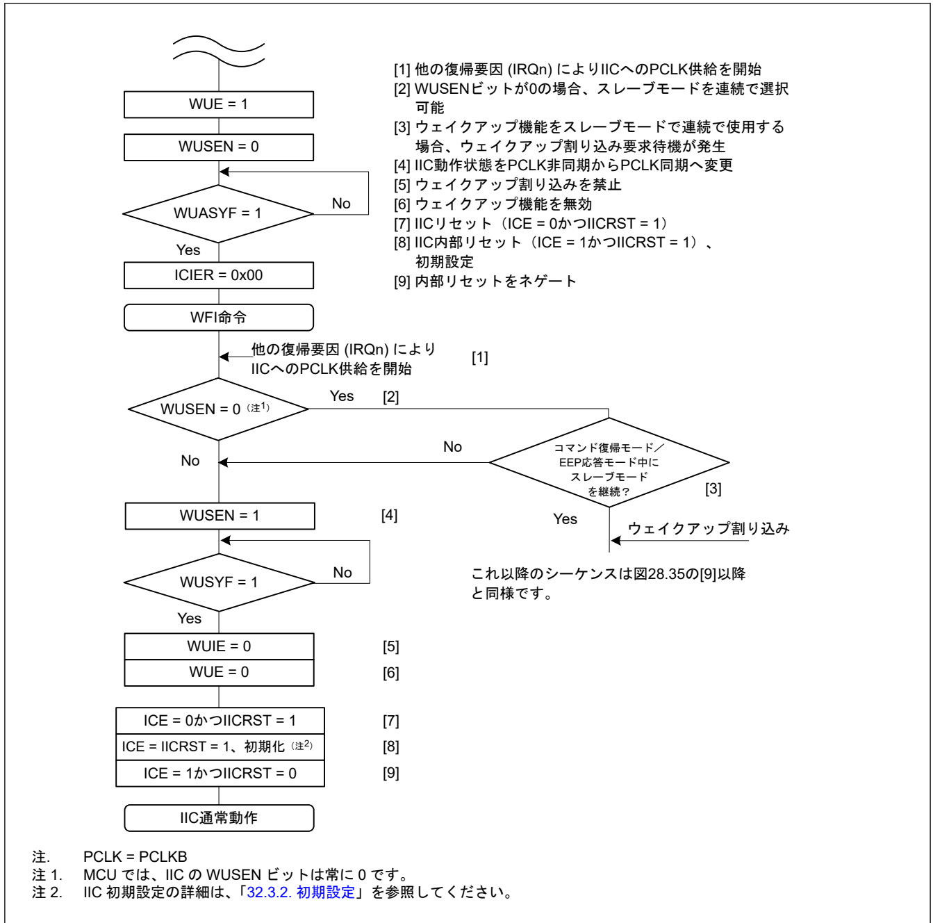
図 32.36 コマンドリカバリモードと EEP 応答モードの動作例 (IIC ウェイクアップ割り込み以外の割り込み (たとえば IRQn) によるウェイクアップの場合)
