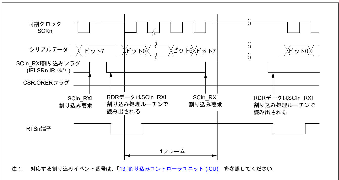
図 31.68 クロック同期式モードにおけるシリアル受信の動作例 (2) (RTS 機能を使用する場合)
