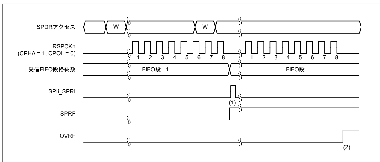
図 36.30 SPCR.TXMD[1:0] = 00b の場合の動作例
