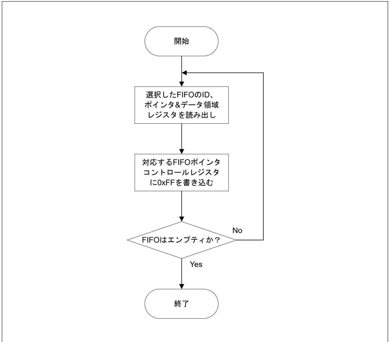
図 34.39 RX FIFO バッファの読み出しフロー（ポーリングの場合の例）
