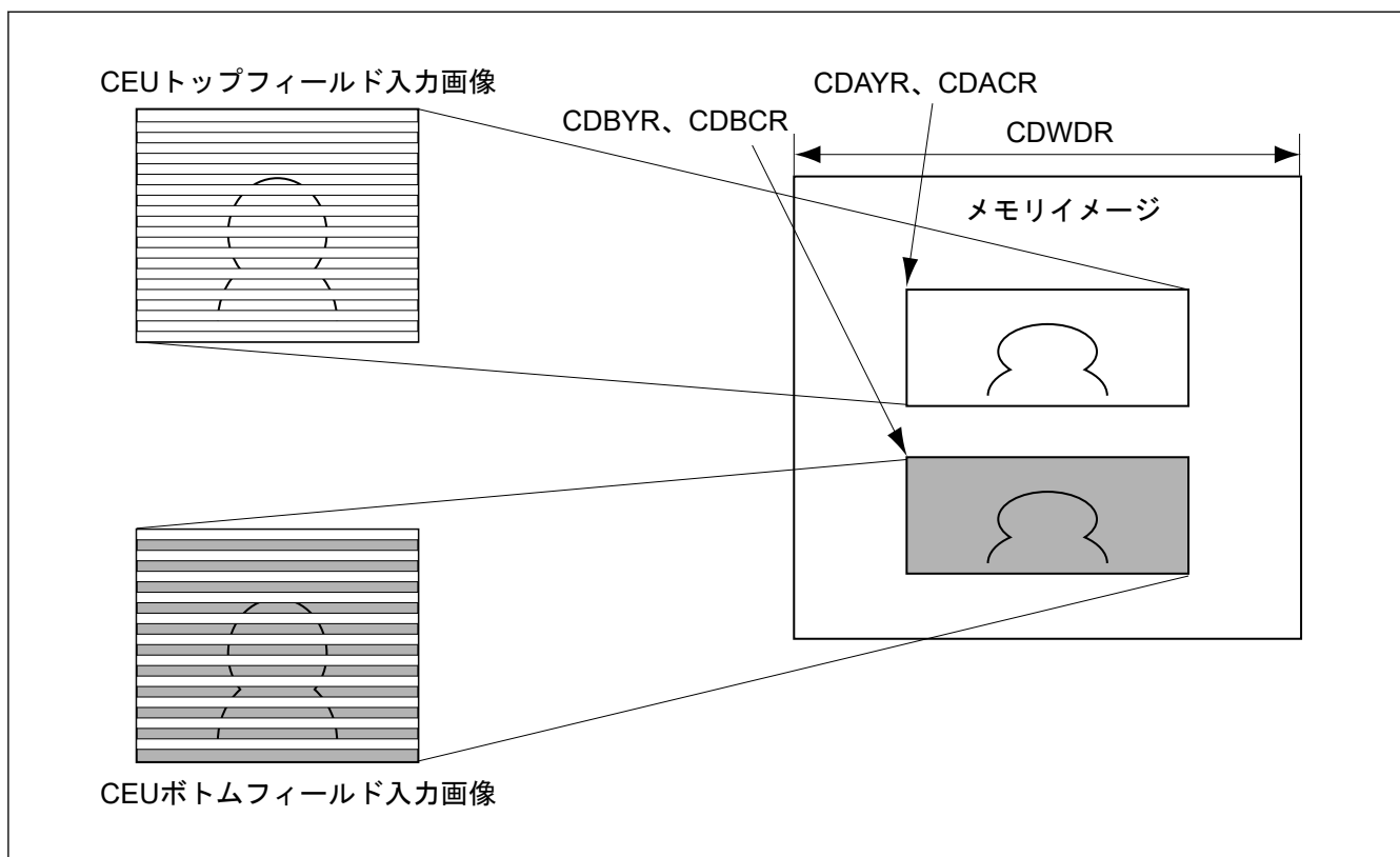
図 53.25 両フィールドキャプチャ画像のメモリ格納イメージ
