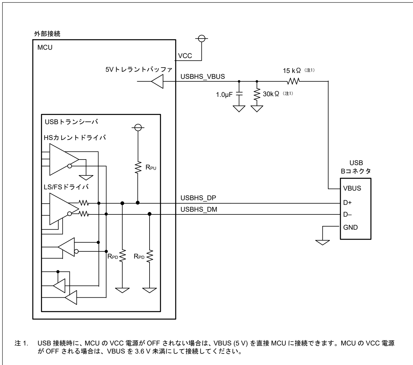
図 30.28 セルフパワーシステムでのデバイス接続例
