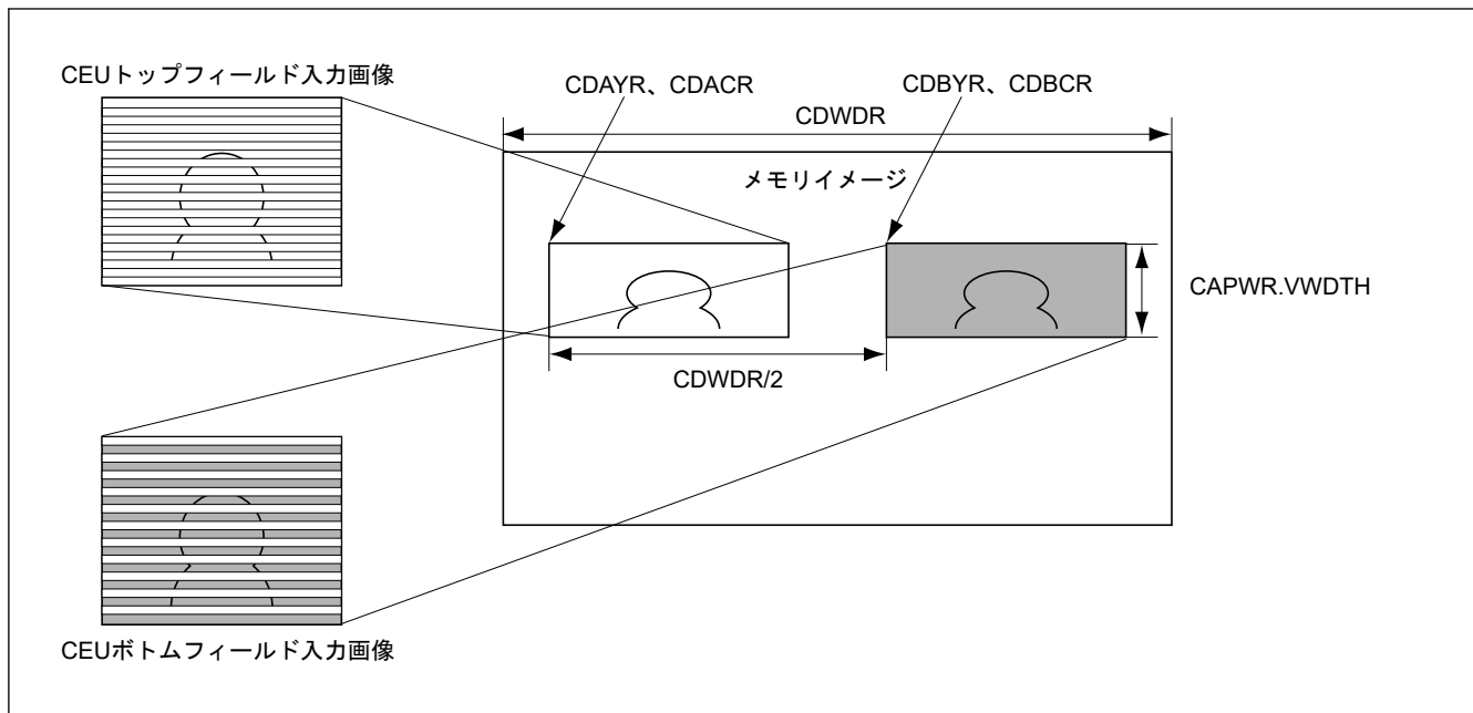
図 53.28 インターレース入力両フィールドキャプチャのメモリ格納イメージ
