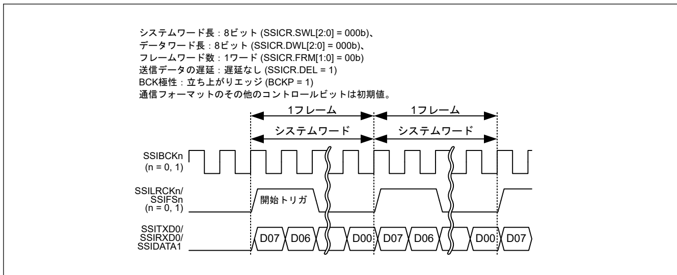
図 39.40 モノラルフォーマットにおけるロングフレーム (パディングなし)
