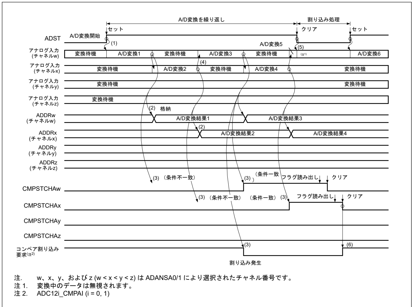
図 45.32 コンペア機能の動作例 (アナログ入力 (チャンネル w~z) を比較)
