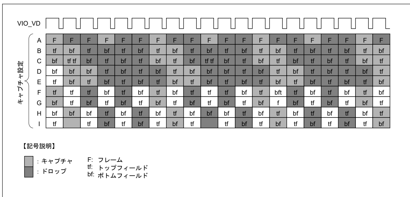
図 53.10 各キャプチャ設定におけるフレームドロップのタイミングイメージ (FDRP[7:0] = 0x2)
