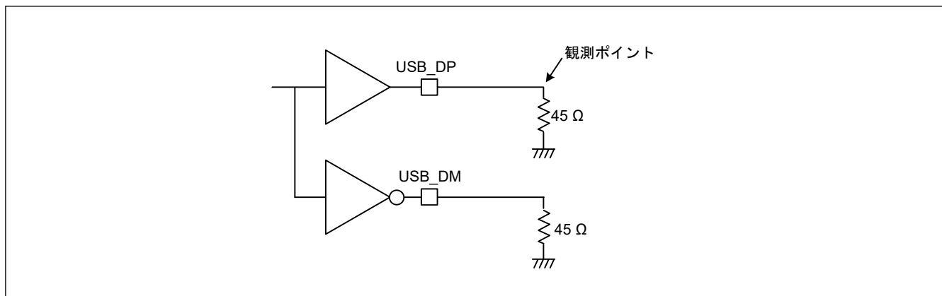
図 55.115 High-speed モードにおける測定回路
