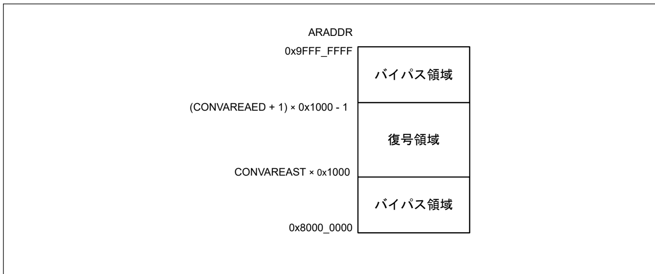
図 38.2 復号領域の設定
