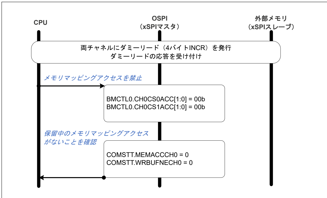
図 37.28 メモリマッピング停止のフロー
