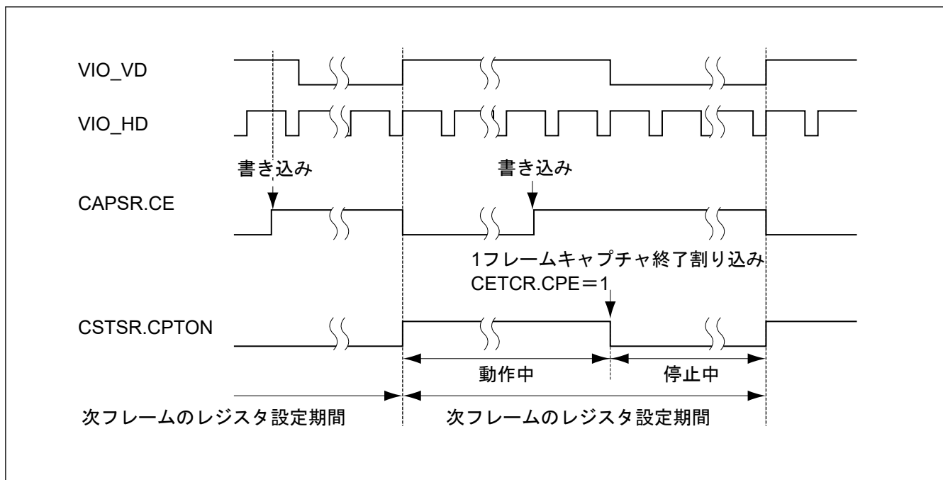
図 53.7 1 フレームキャプチャの CE ビット書き込みタイミングとレジスタ設定
