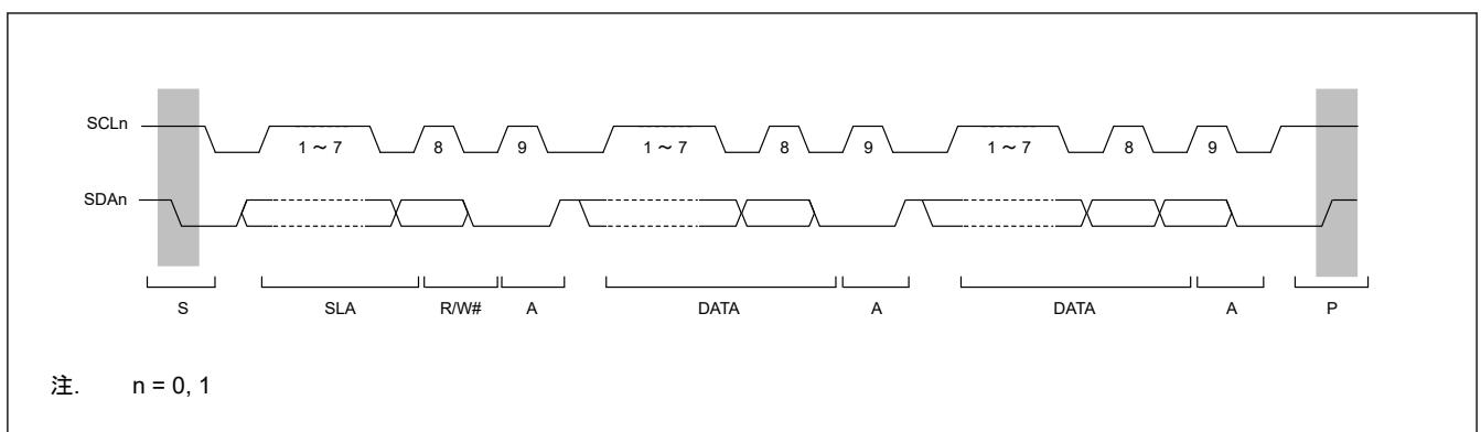
図 32.4 I2C パスタイミング (SLA = 7 ビットの場合)
