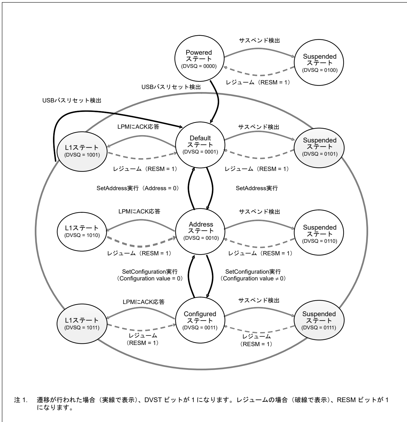
図 30.8 デバイスステートの遷移
