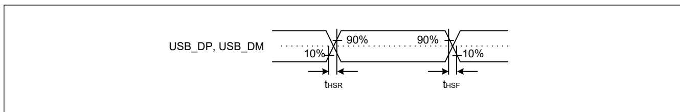
図 55.114 High-speed モードにおける USB_DP、USB_DM の出力タイミング
