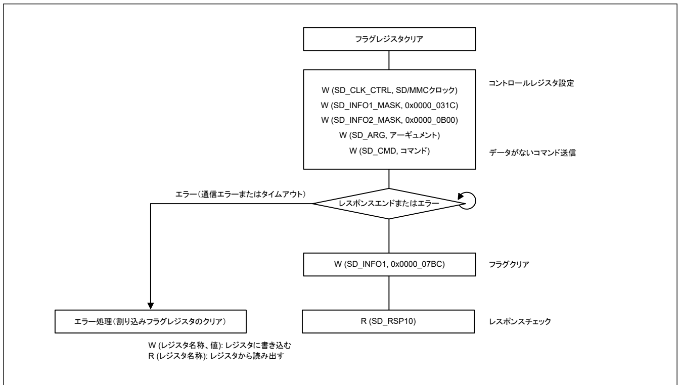
図 40.10 データがないコマンドのフロー例
