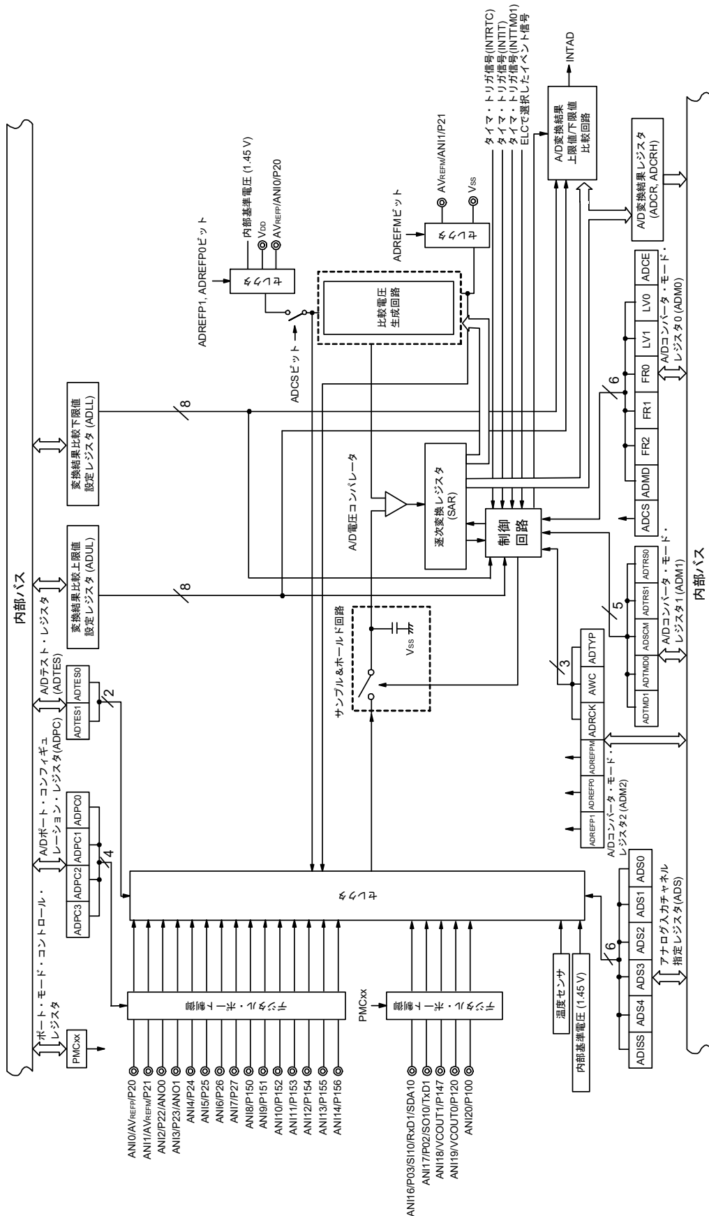
図14-1 A/Dコンバータのブロック図
