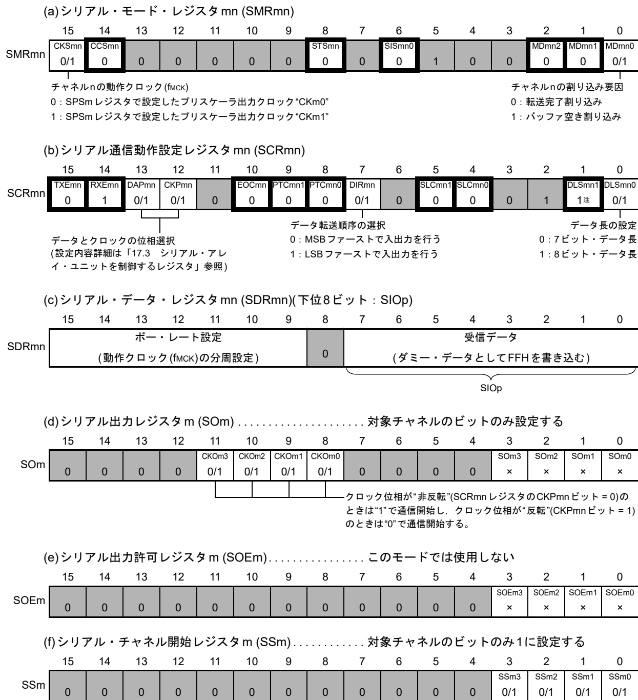
図 17 - 36 簡易SPI (CSI00, CSI01, CSI10, CSI11, CSI20, CSI21, CSI30, CSI31)のマスター受信時のレジスタ設定内容例
