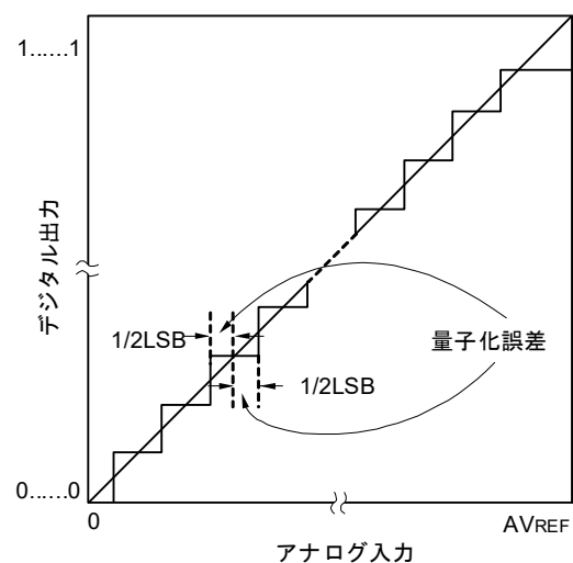
図14-41 量子化誤差
