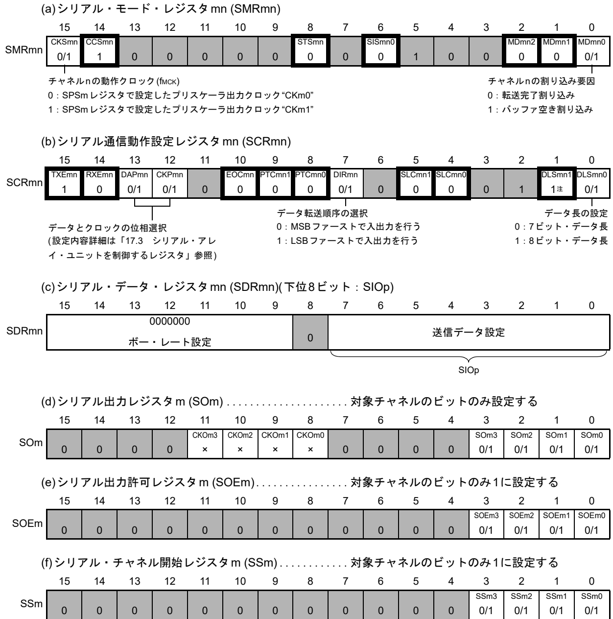
図 17 - 52 簡易SPI (CSI00, CSI01, CSI10, CSI11, CSI20, CSI21, CSI30, CSI31)のスレーブ送信時のレジスタ設定内容例
