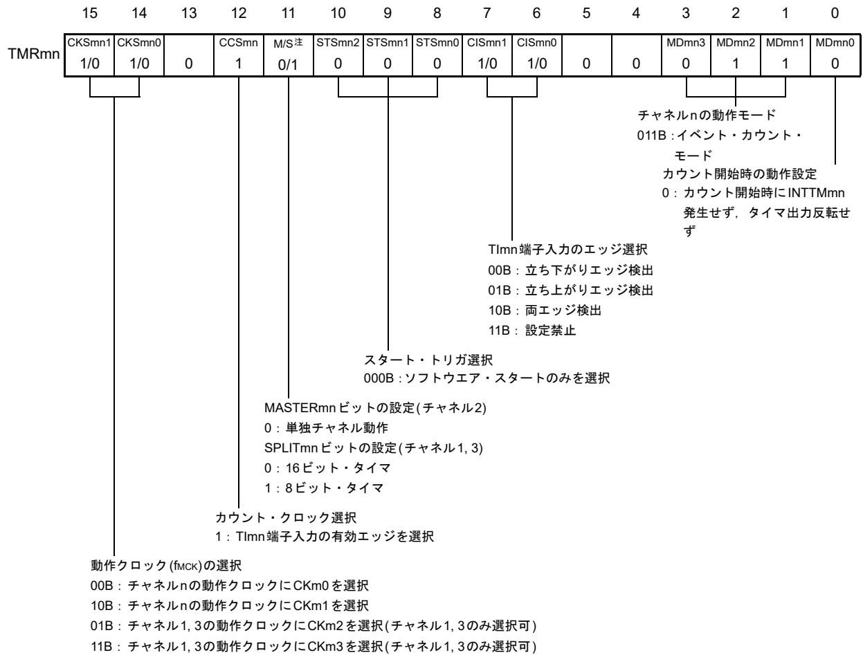
図6 - 53 外部イベント・カウンタ・モード時のレジスタ設定内容例
