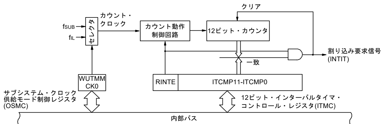
図 11 - 1 12ビット・インターバル・タイマのブロック図
