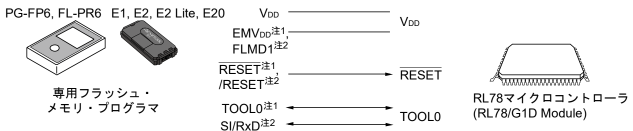
図3-2 専用フラッシュ・メモリ・プログラマとの通信
