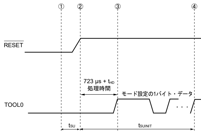
図3-7 フラッシュ・メモリ・プログラミング・モードへの引き込み
