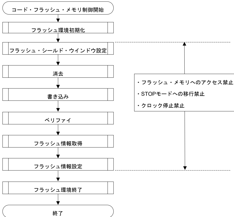
図3-8 セルフ・プログラミング（フラッシュ・メモリの書き換え）の流れ
