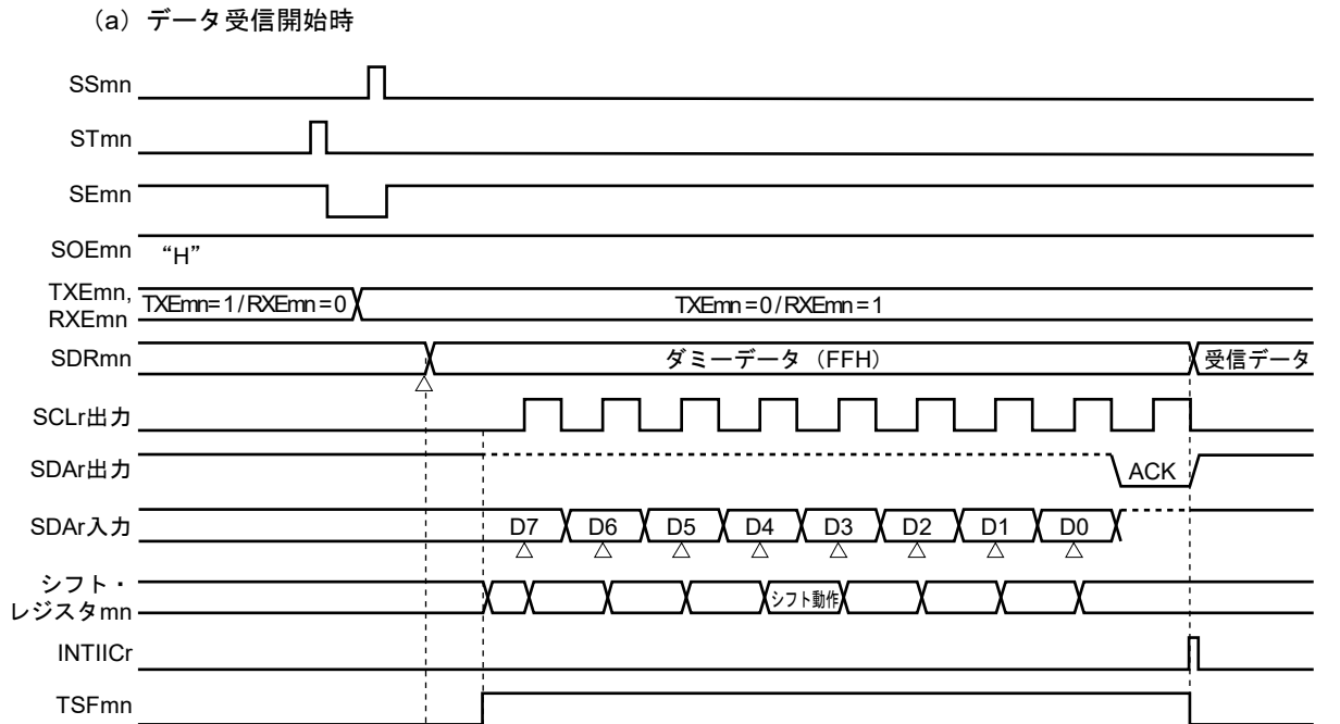
図18-111 データ受信のタイミング・チャート
