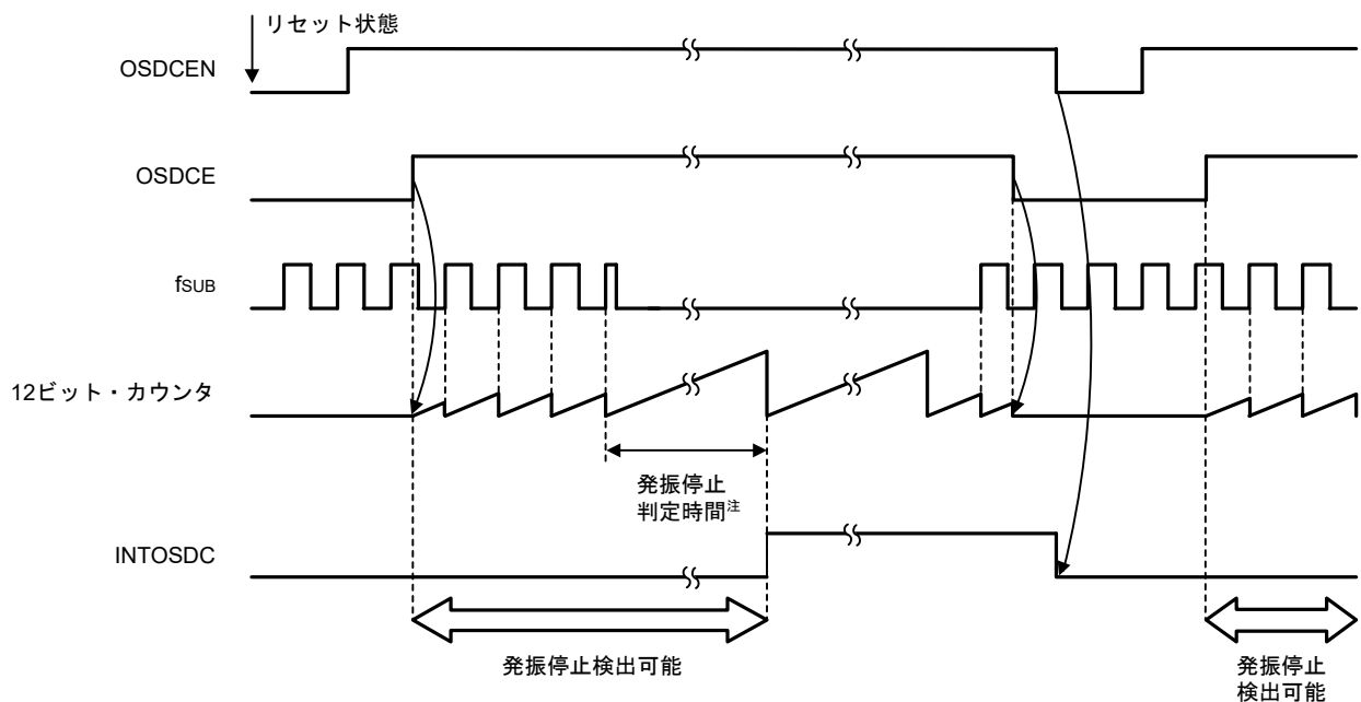
図29-5 発振停止検出回路のタイミング
