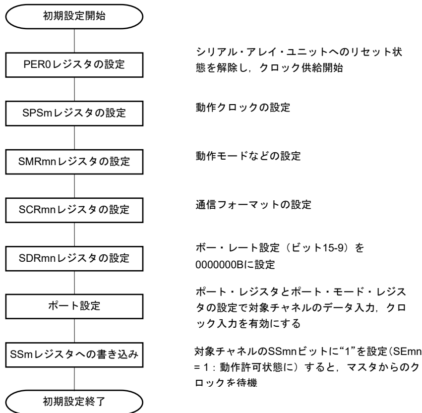
図18-58 スレーブ受信の初期設定手順
