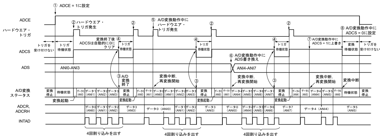
図14-28 ハードウェア・トリガ・ウエイト・モード (スキャン・モード, ワンショット変換モード) 動作タイミング例
