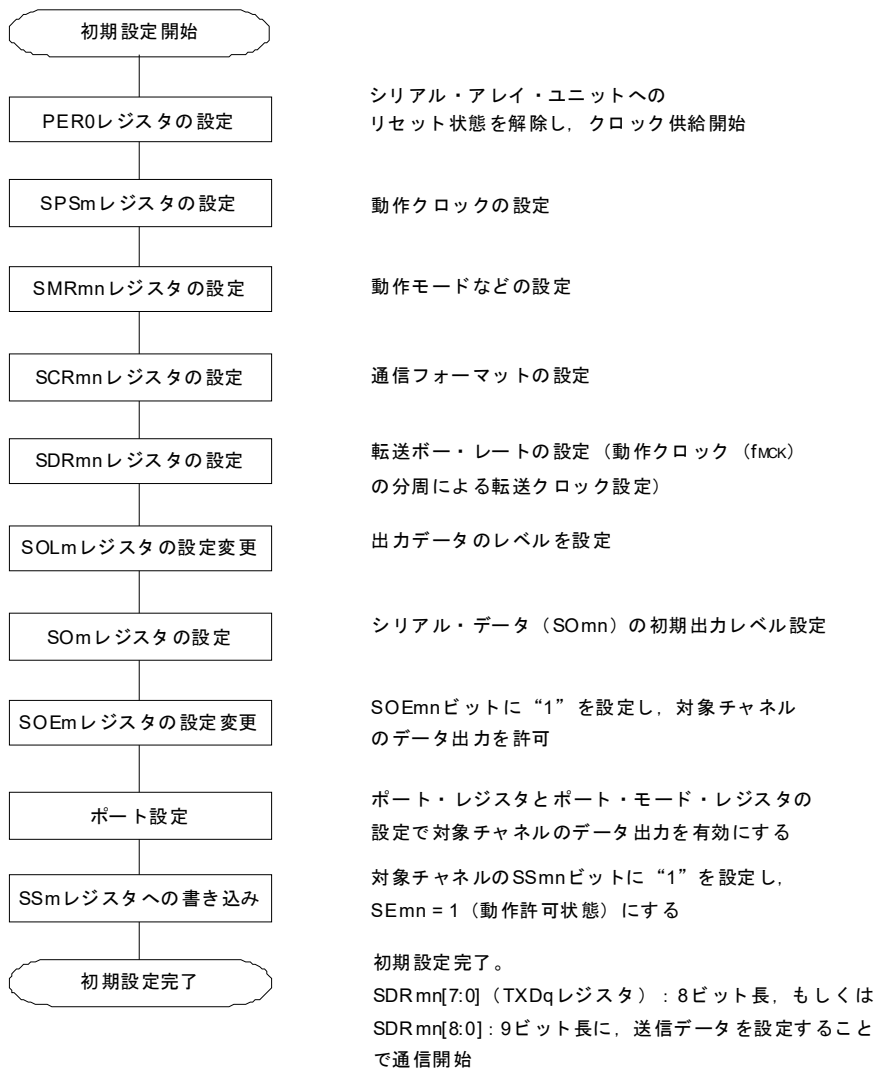
図18-77 UART送信の初期設定手順
