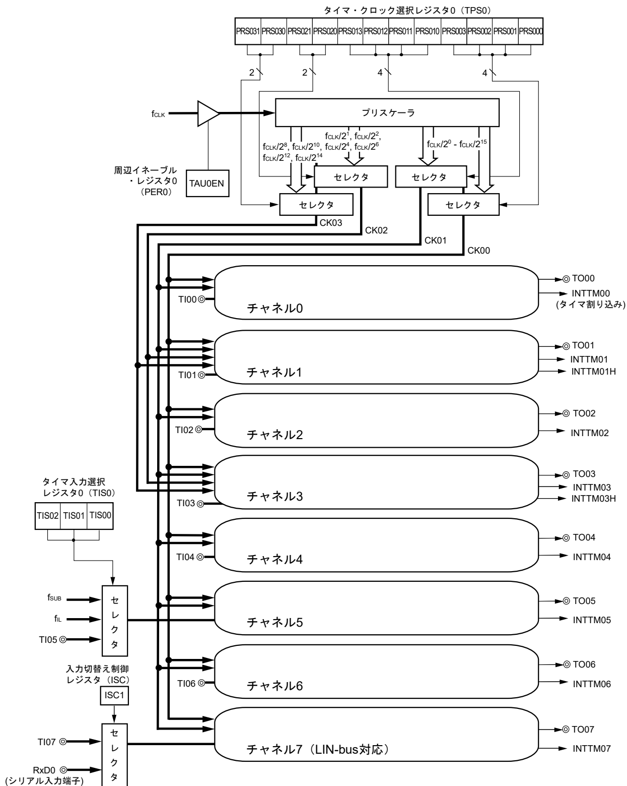
図7-1 タイマ・アレイ・ユニットの全体ブロック図
