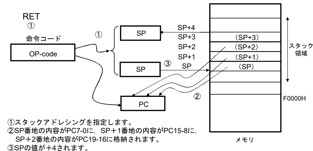
図3-36 RETの例
