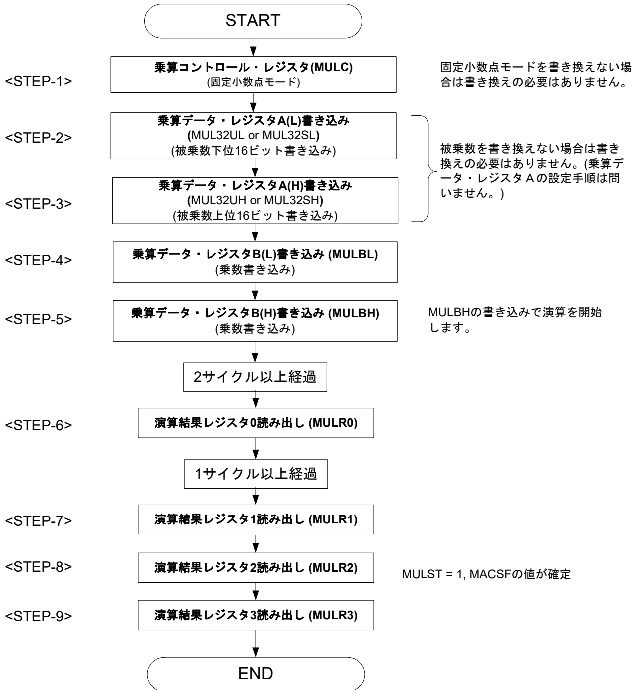
図39-8 32ビット積和演算回路の動作フロー（乗算時）
