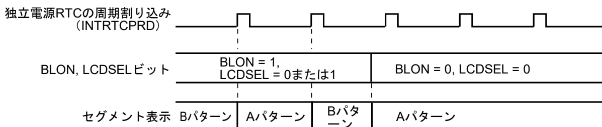
図21-15 点滅表示からAパターン表示への切り替え動作
