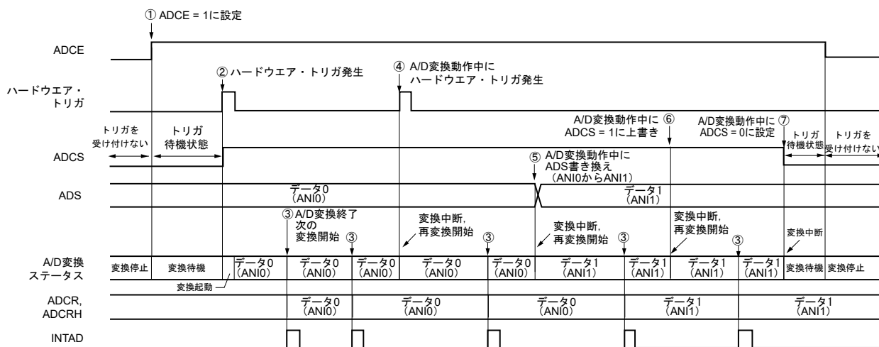
図15-26 ハードウェア・トリガ・ウエイト・モード (セレクト・モード, 連続変換モード) 動作タイミング例
