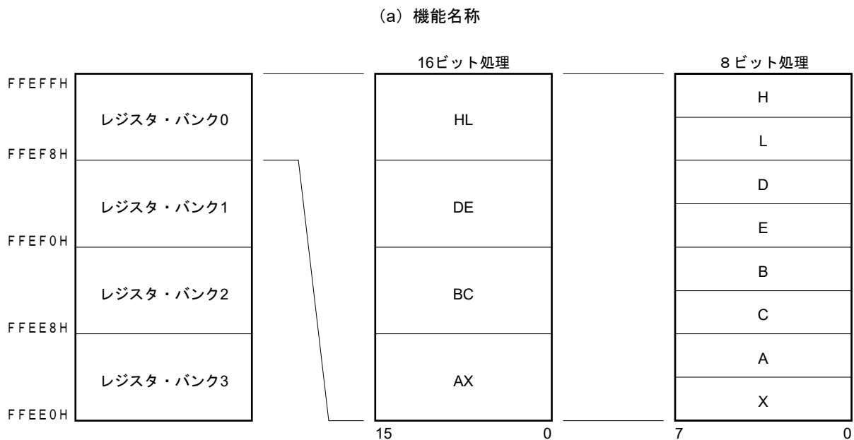
図3-9 汎用レジスタの構成
