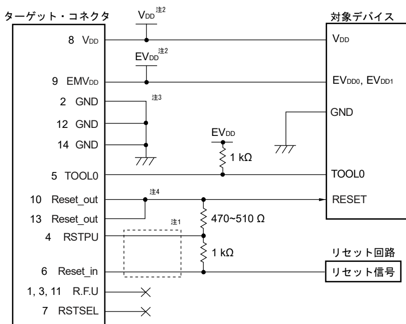
図37-2 E1オンチップデバッキングエミュレータとの接続例(バッテリーバックアップ機能を使用しない場合)
