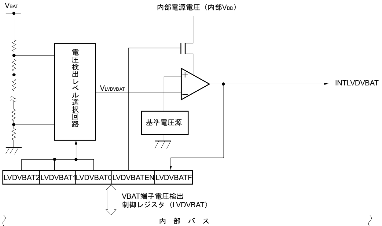
図29-3 V BAT 端子電圧検出回路のブロック図
