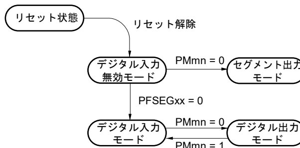
図21-11 SEGxx/Pxx端子機能の状態遷移図
