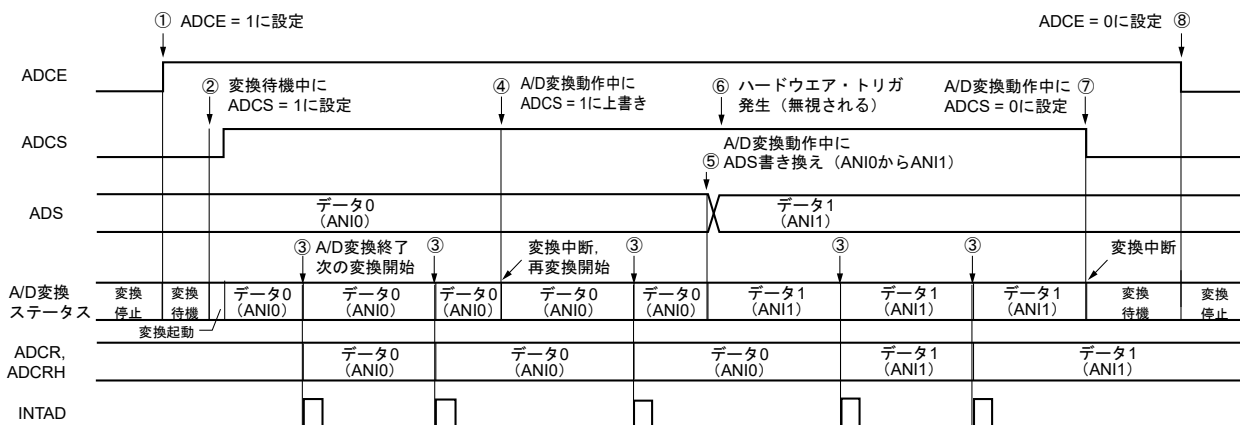
図15-18 ソフトウェア・トリガ・モード（セレクト・モード，連続変換モード）動作タイミング例
