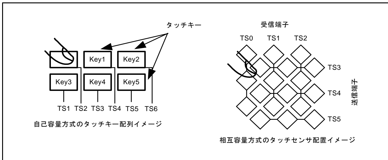
図 32.12 自己容量方式と相互容量方式の概要
