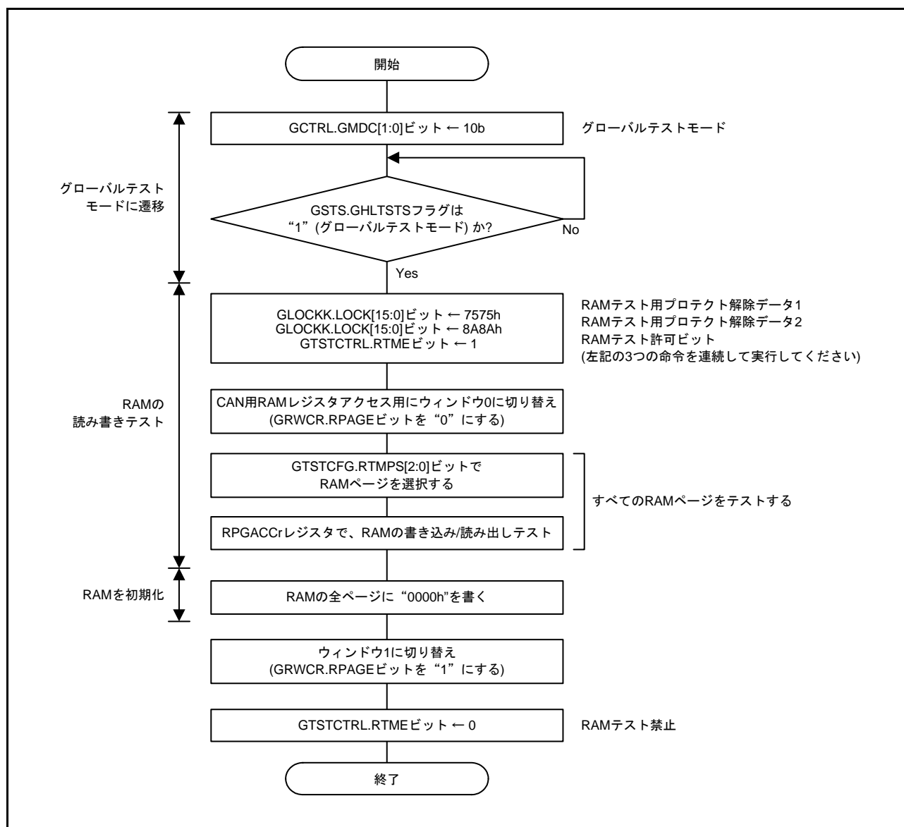
図 29.35 RAMテストの設定手順
