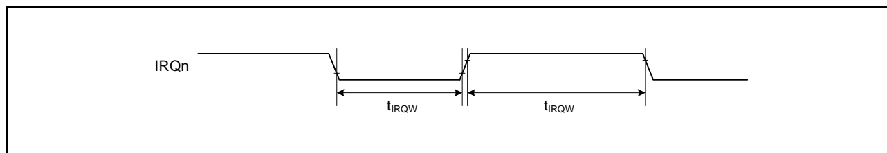
図 42.28 IRQ 割り込み入力タイミング
