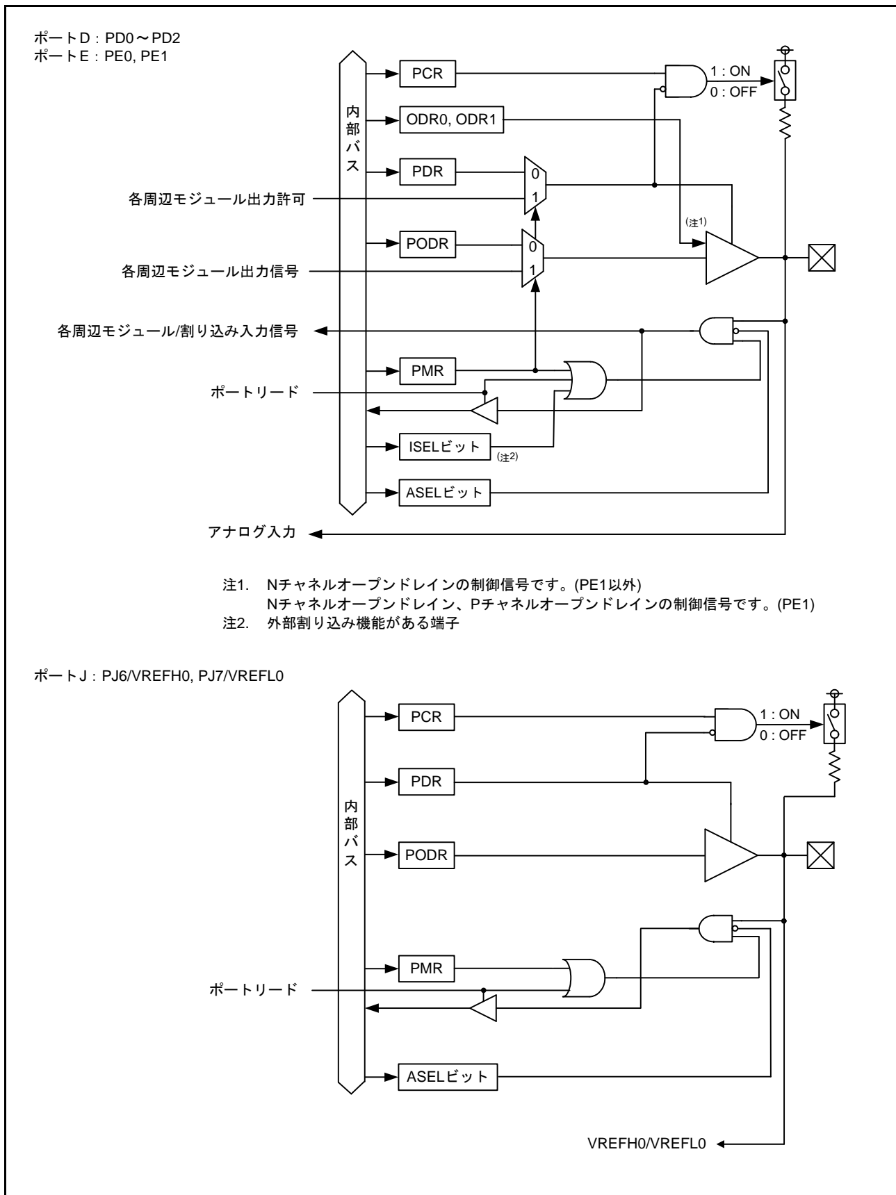
図 18.7 入出力ポートの構成 (7)
