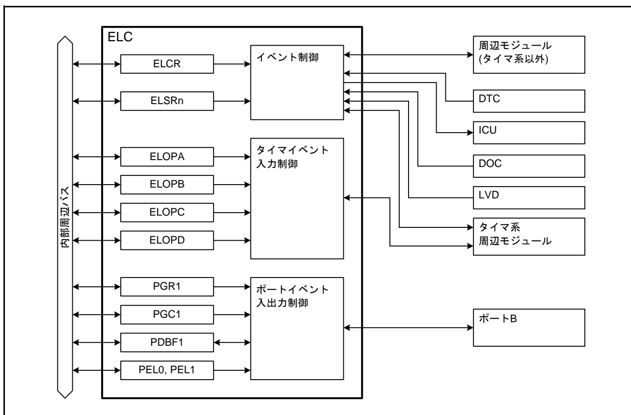
図 17.1 ELC のブロック図 (n = 1 ~ 4, 7, 8, 10, 12, 14 ~ 16, 18, 20, 22, 24, 25)
