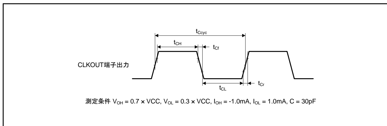
図 42.53 CLKOUT 出力タイミング
