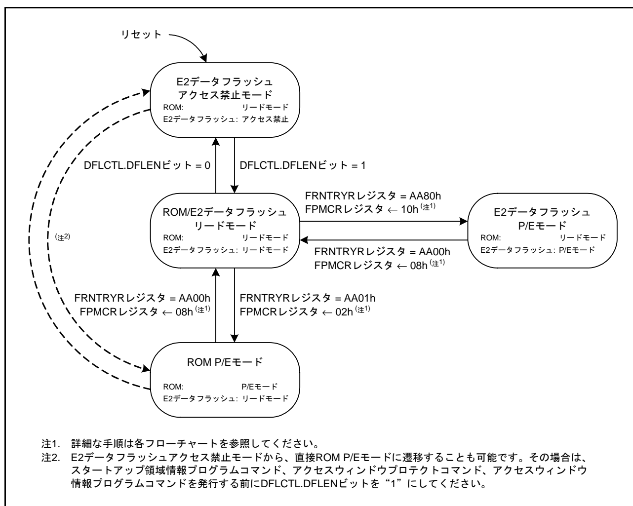
図 41.6 フラッシュメモリのモード移行図
