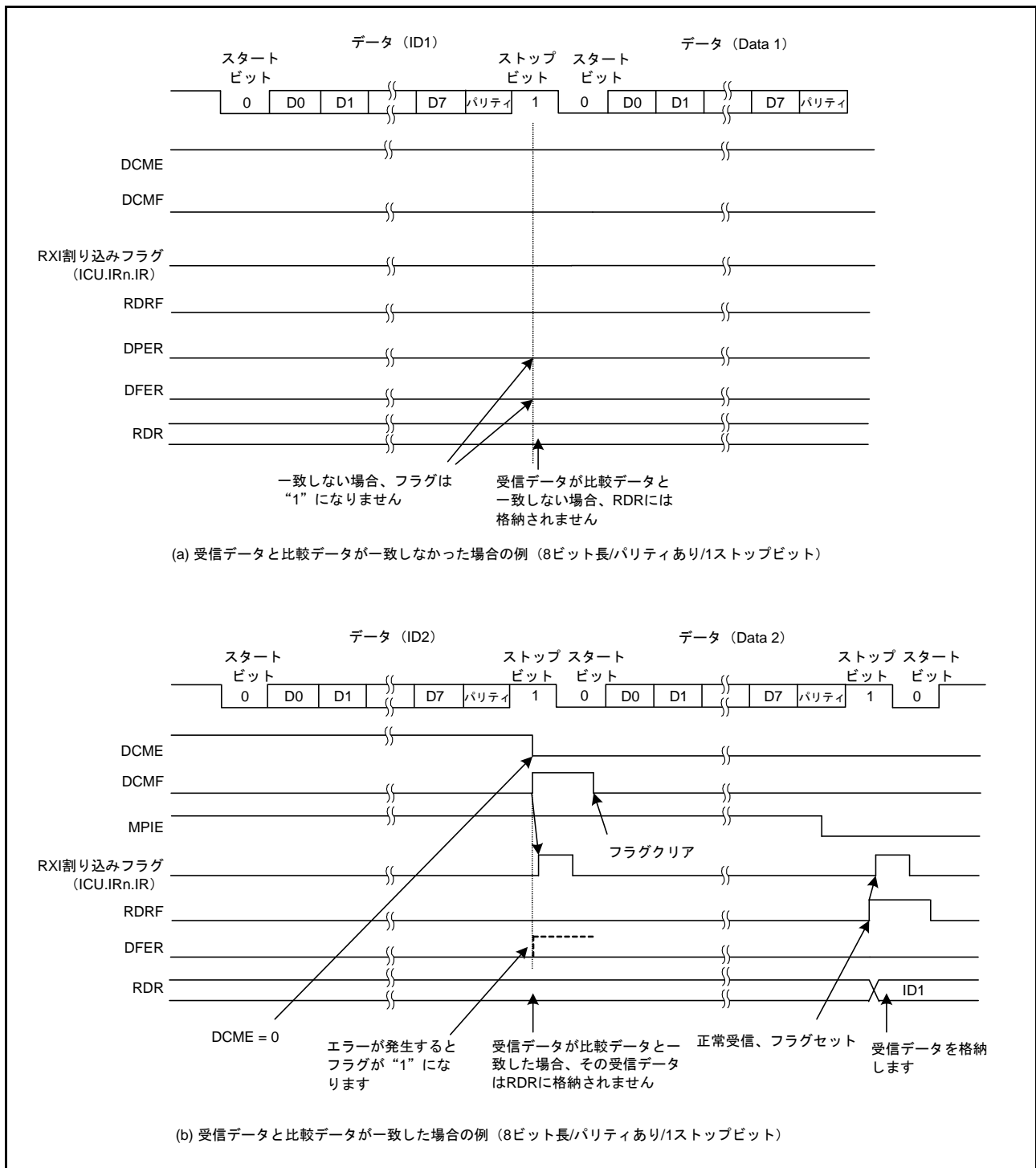
図 27.10 データ一致検出の例 (1) 非マルチプロセッサモード
