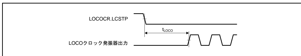
図 42.16 LOCO クロック発振開始タイミング
