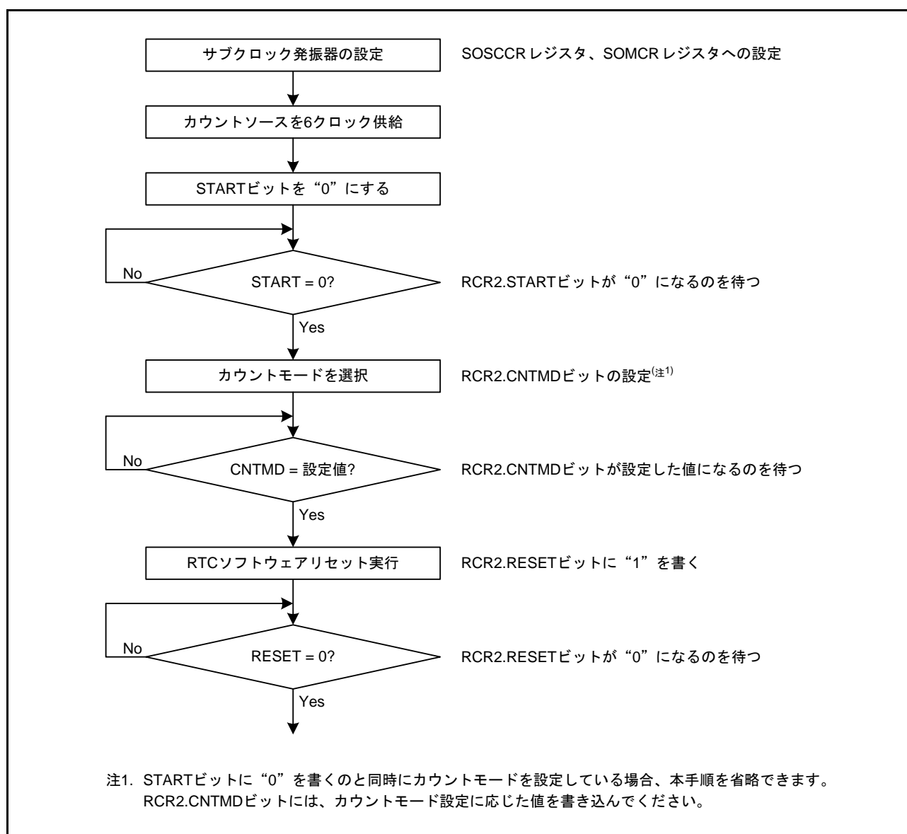
図 24.3 クロック設定手順
