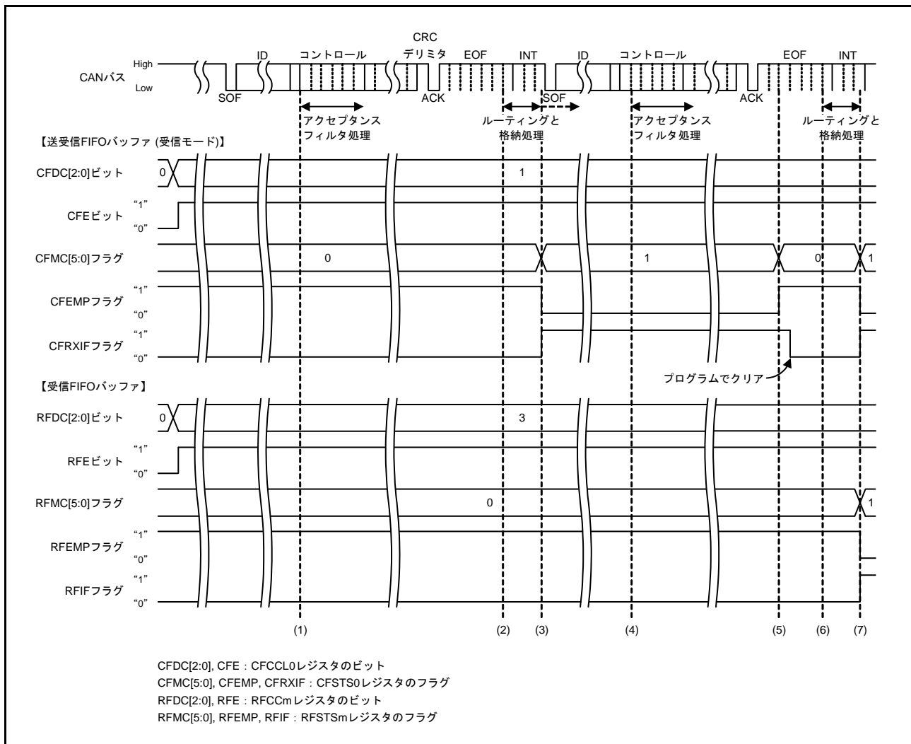
図 29.25 FIFO バッファの受信タイミング図
