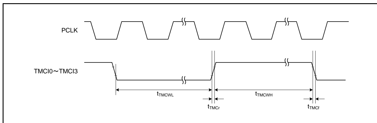
図 42.37 TMR クロック入力タイミング
