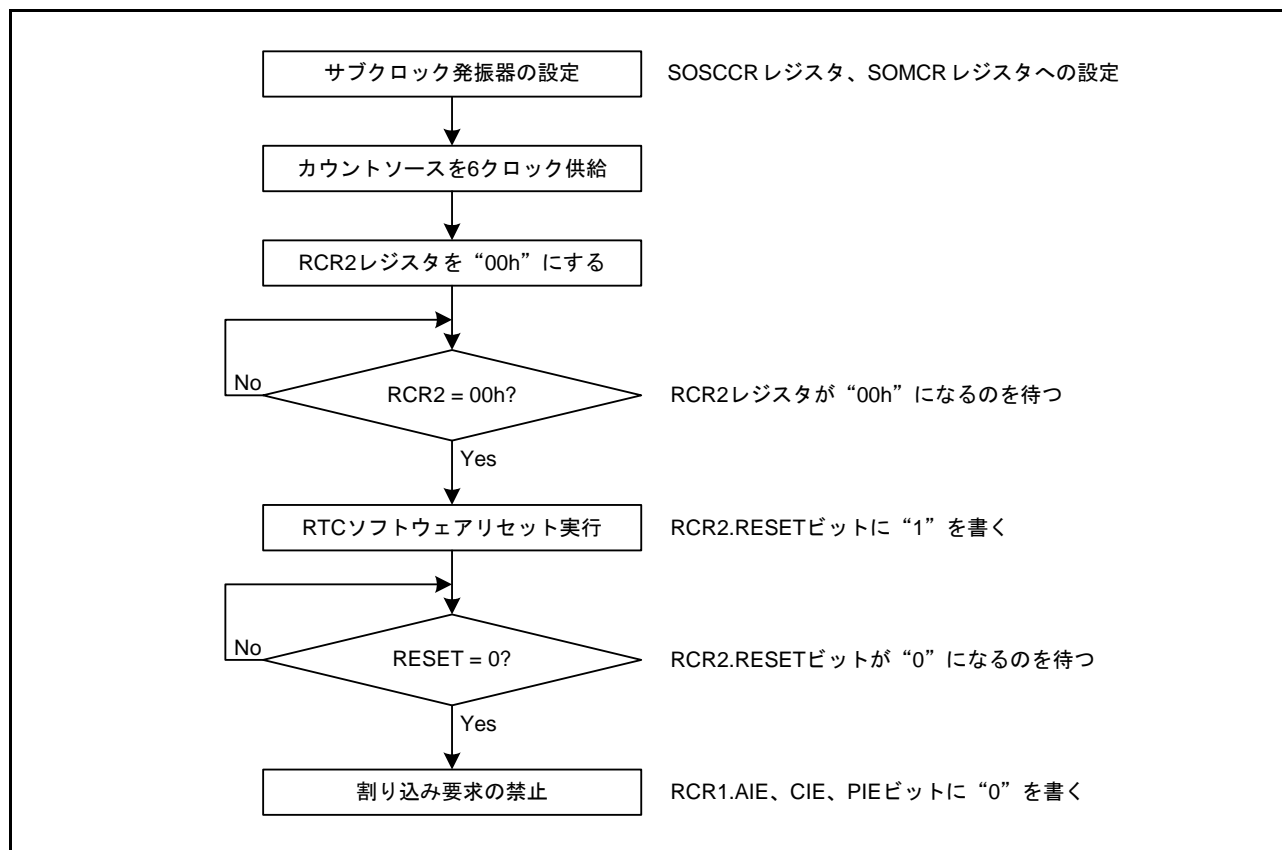
図 24.12 初期化手順
