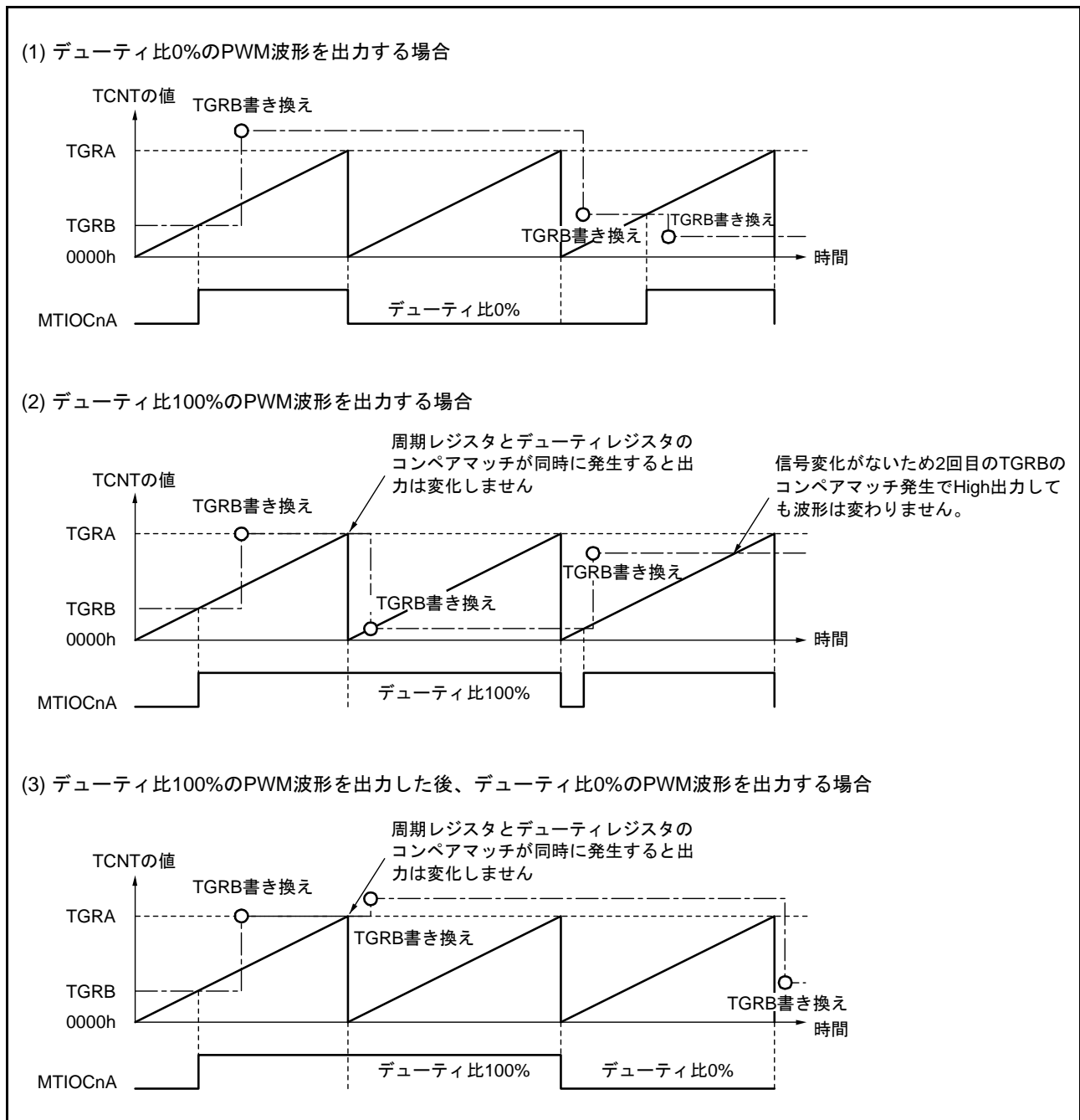
図 20.28 PWMモード動作例 (デューティ0%、デューティ100%のPWM波形を出力する例) ( n = 0 \sim 4 )
