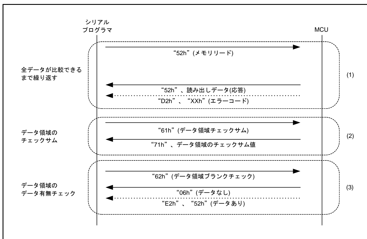
図 41.38 データ領域のデータ確認手順
