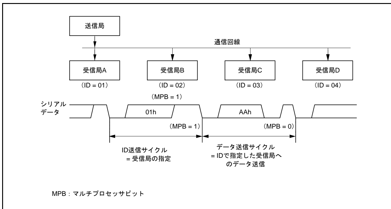
図 27.22 マルチプロセッサフォーマットを使用した通信例 (受信局 A へのデータ“AAh”の送金の例)
