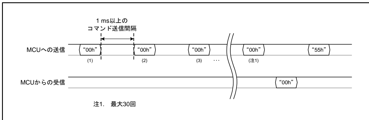
図 41.29 ビットレート自動調整時のデータフォーマット
