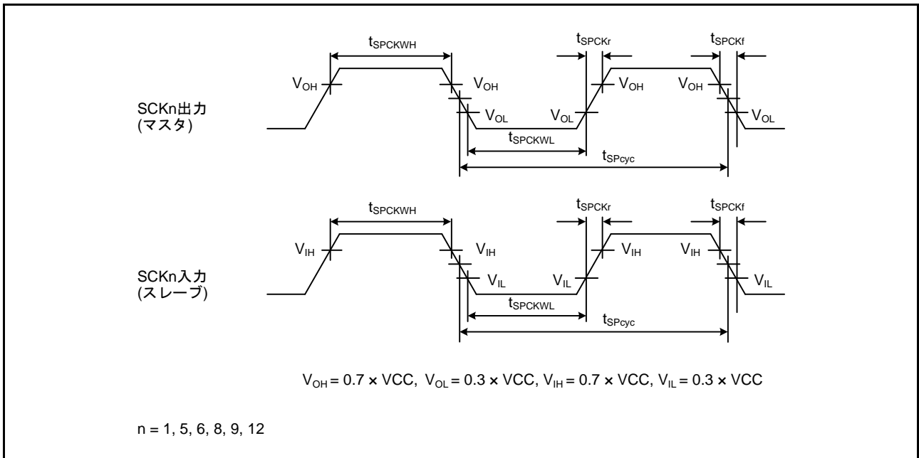
図 42.41 簡易 SPI クロックタイミング
