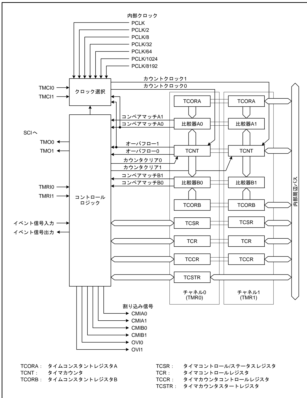
図 22.1 TMR (ユニット0) のブロック図
