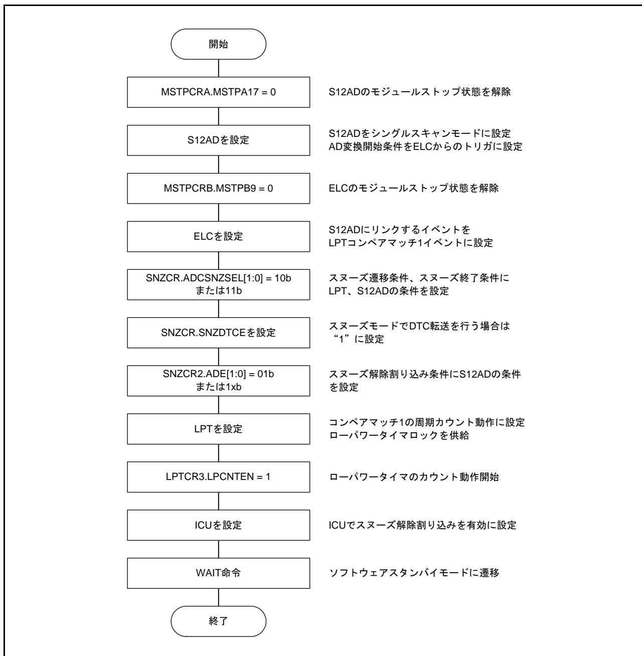
図 11.12 スleepモードでの S12AD 変換動作設定フローの例
