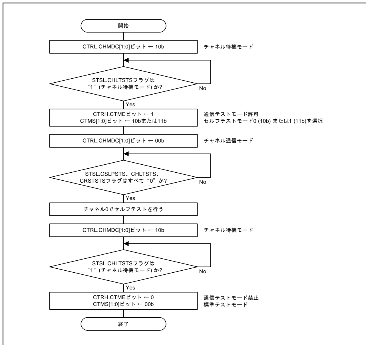
図 29.33 セルフテストモードの設定手順
