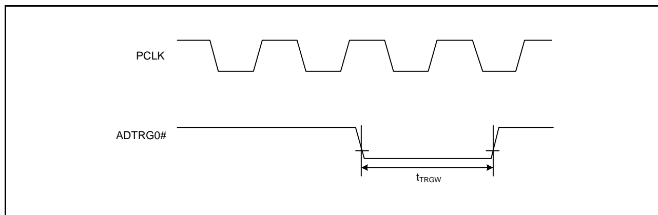
図 42.52 A/Dコンバータ外部トリガ入力タイミング
