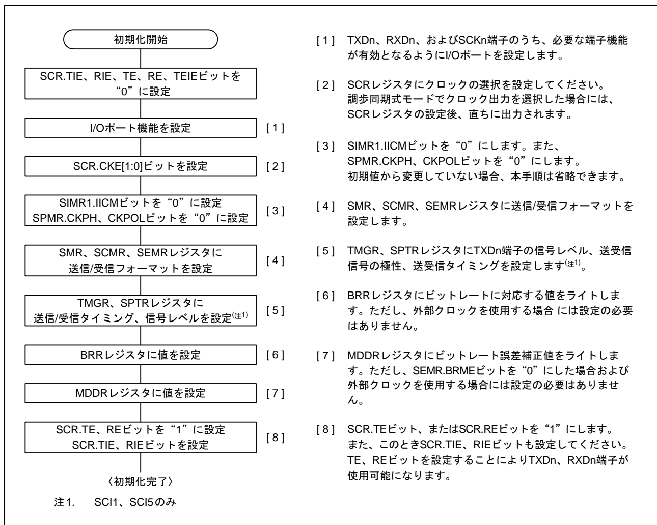
図 27.12 SCIの初期化フローチャートの例 (調歩同期式モード)
