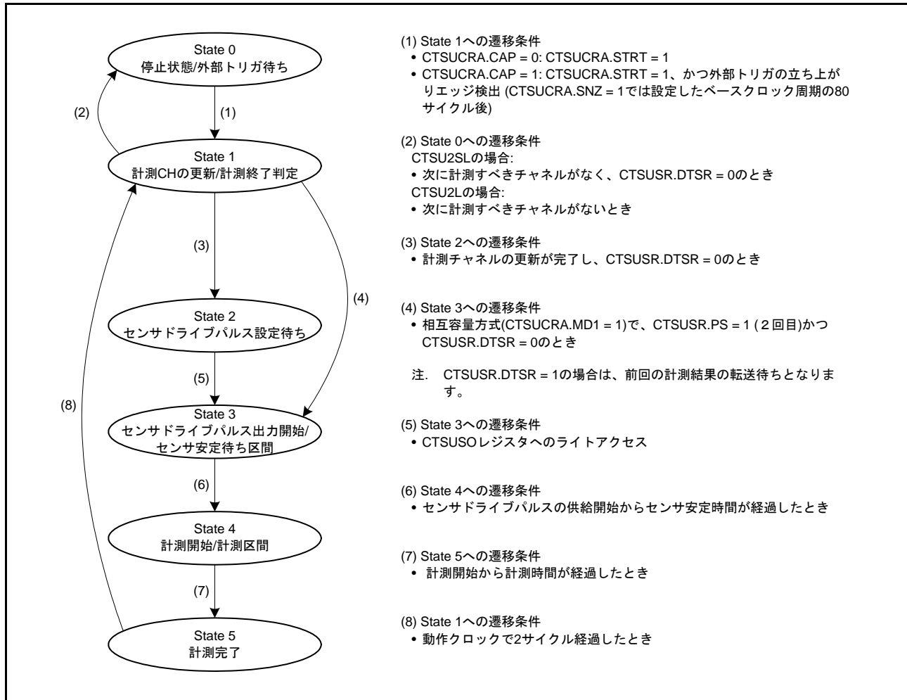
図 32.11 状態遷移図
