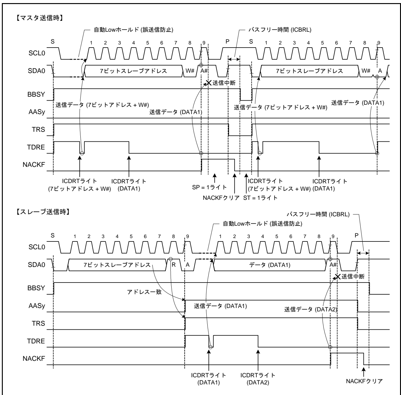
図 28.30 NACK 受信時の転送中断動作 (NACKF ビット = 1 のとき)
