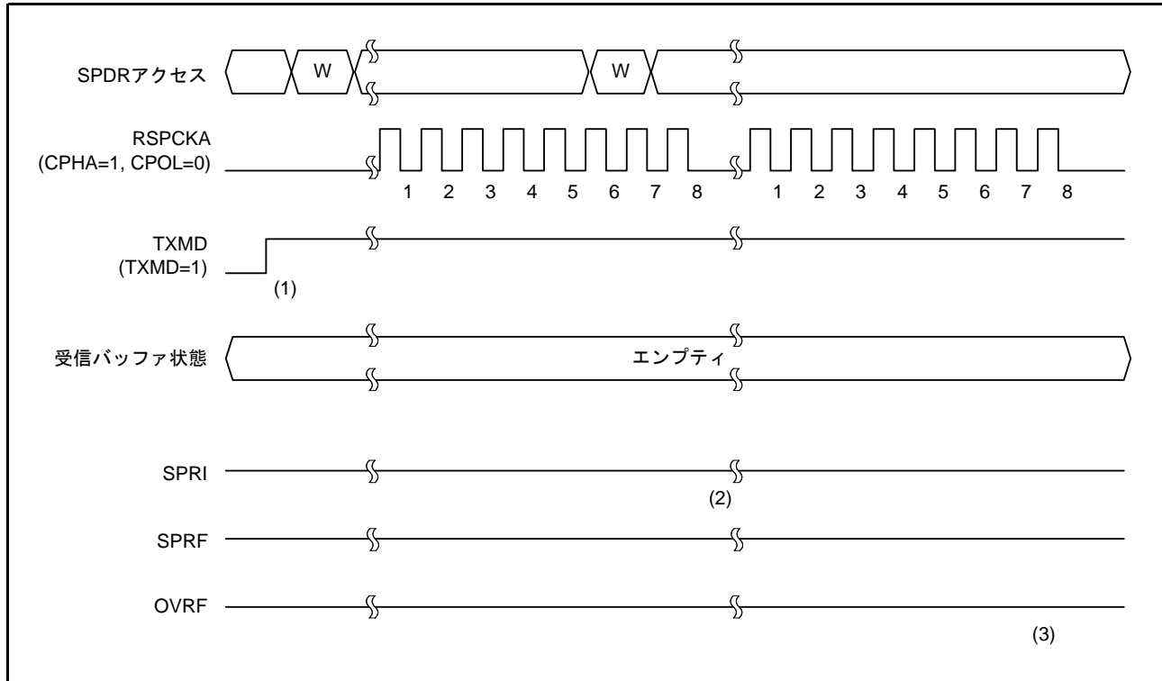
図 30.27 SPCR.TXMD = 1 の動作例
