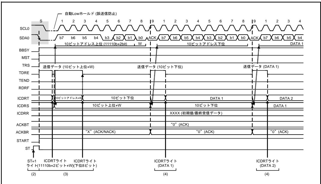
図 28.7 マスタ送信の動作タイミング (2) (10ビットアドレスフォーマットの時)
