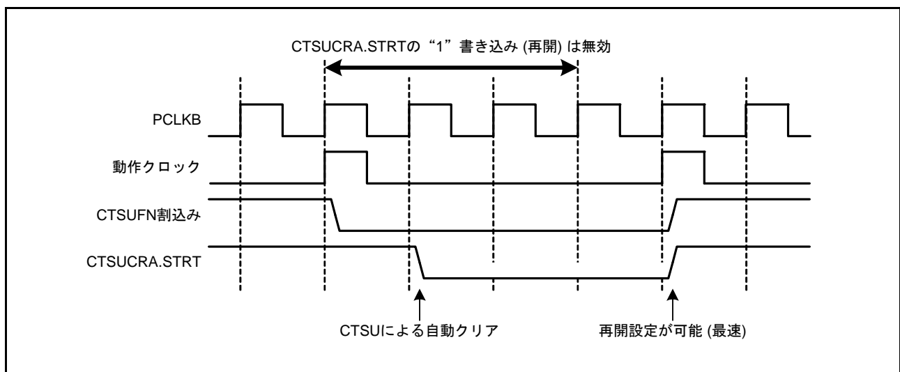
図 32.15 再開時の注意事項
