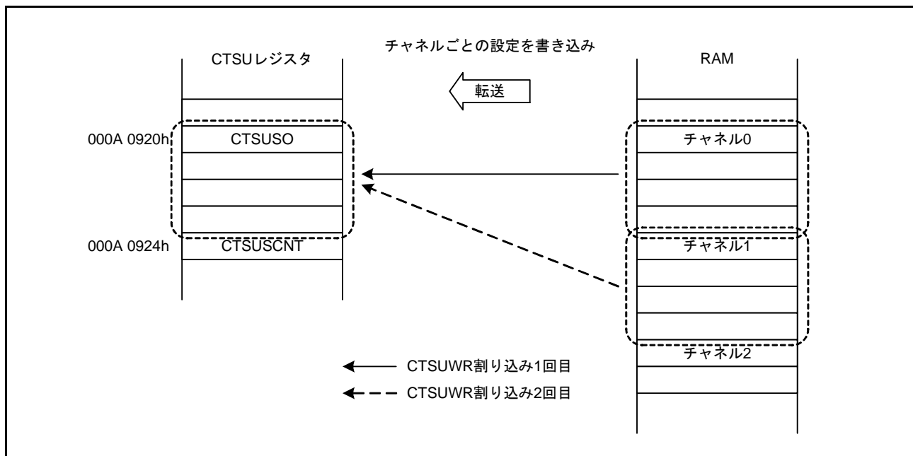
図 32.13 CTSUSWR 割り込みを用いた DTC 転送動作例
