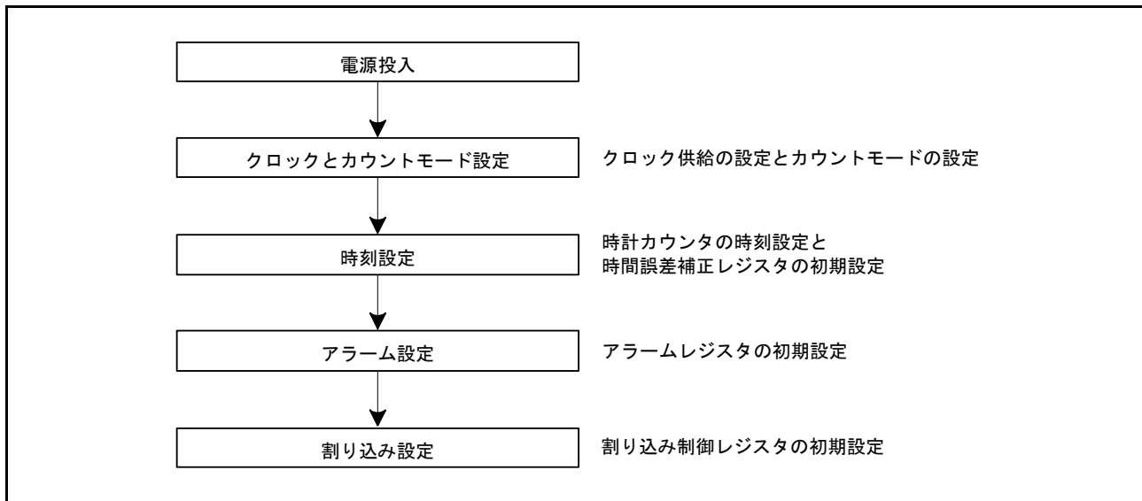
図 24.2 電源投入後の初期設定概要
