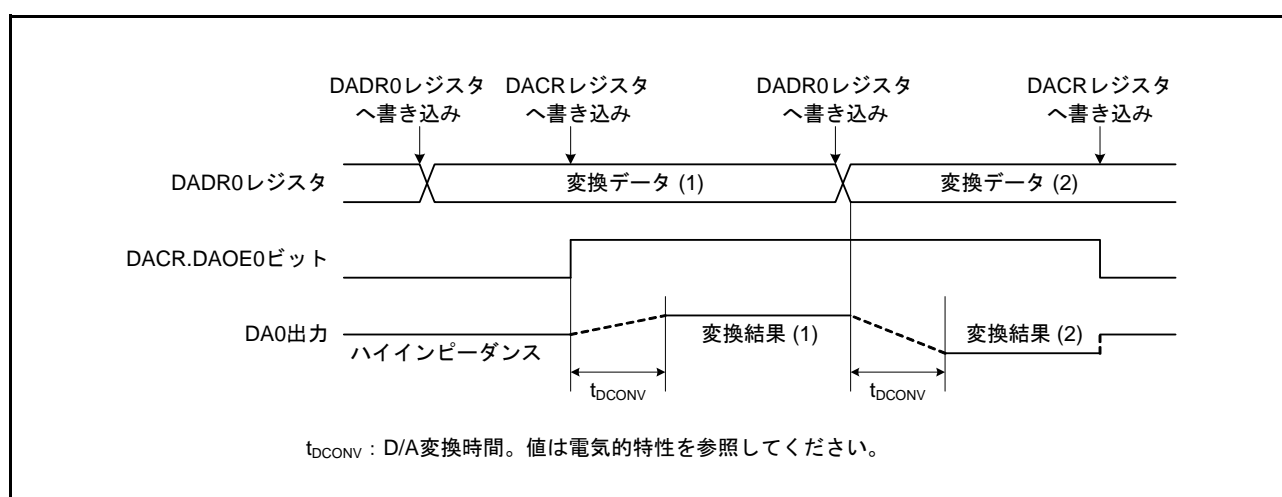
図 36.2 8ビットD/Aコンバータの動作例
