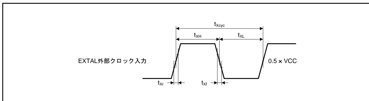
図 42.14 EXTAL 外部クロック入力タイミング
