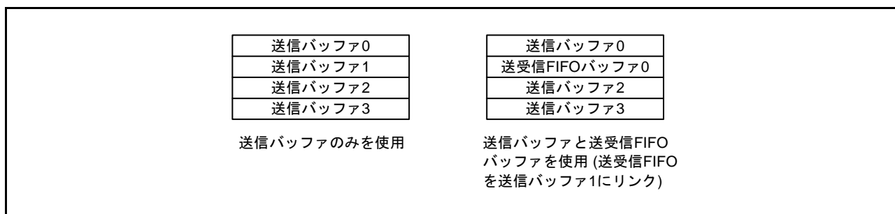
図 29.7 送受信 FIFO バッファのリンク
