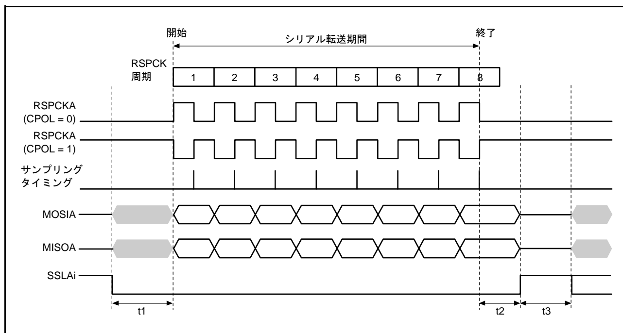
図 30.25 RSPI 転送フォーマット (CPHA ビット = 1)
