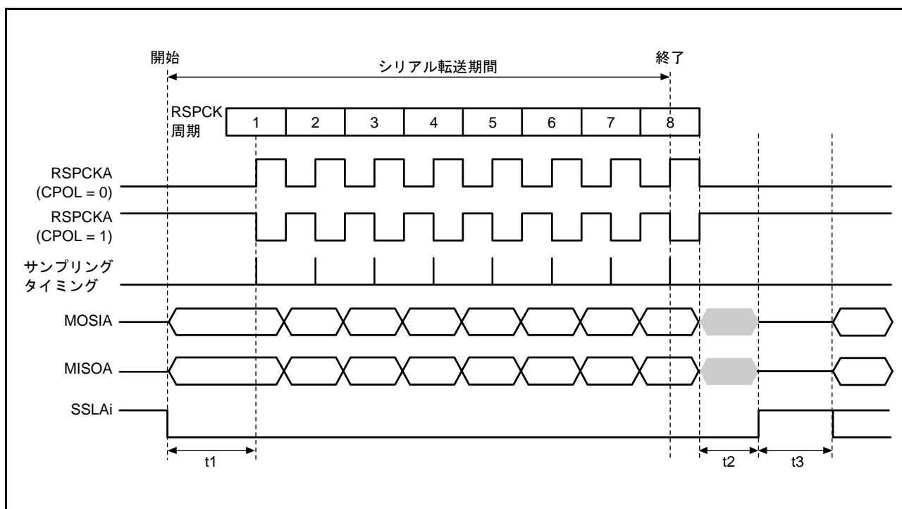
図 30.24 RSPI 転送フォーマット (CPHA ビット = 0)
