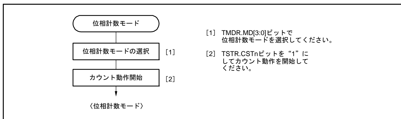
図 20.29 位相計数モードの設定手順例
