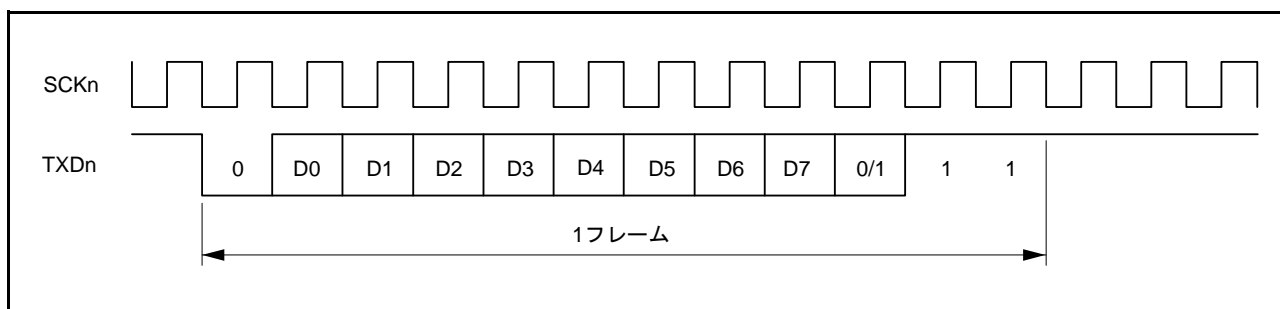
図 27.9 出カクロックと送信データの位相関係 (調歩同期式モード: SMR.CHR = 0、PE = 1、MP = 0、STOP = 1)
