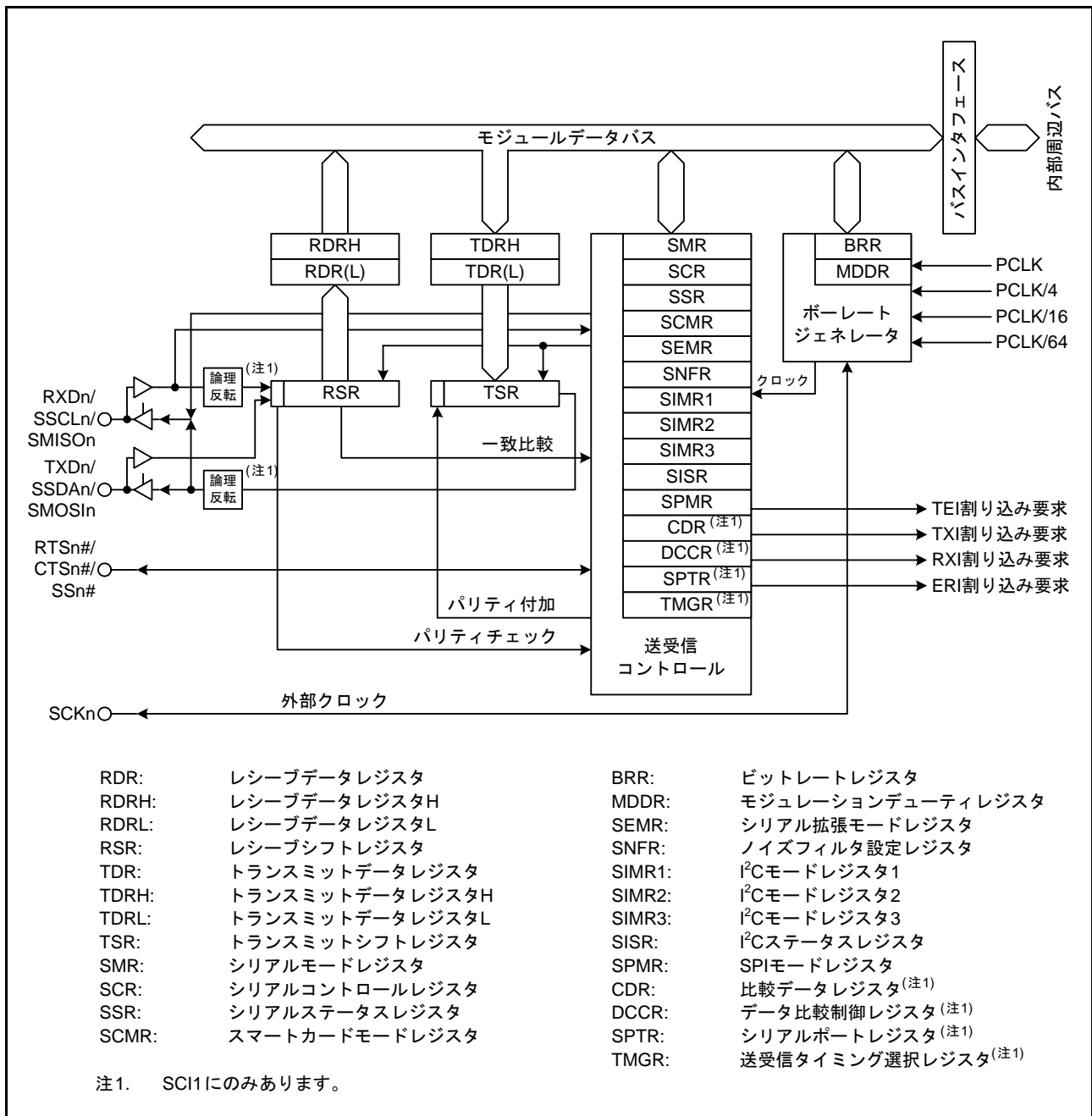
図 27.1 SCIg, SCIk (SCI1, SCI8, SCI9) のブロック図
