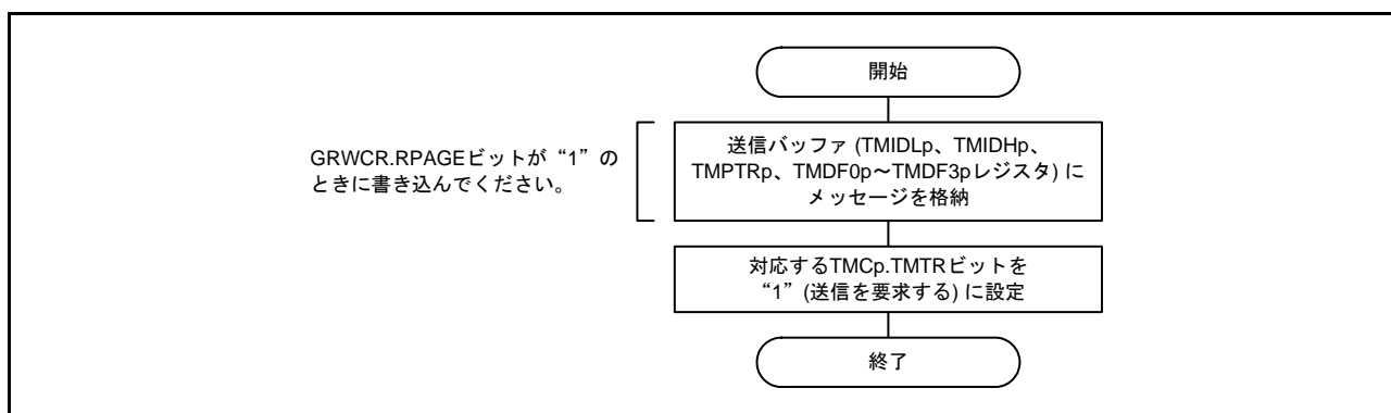
図 29.26 送信バッファからの送信手順
