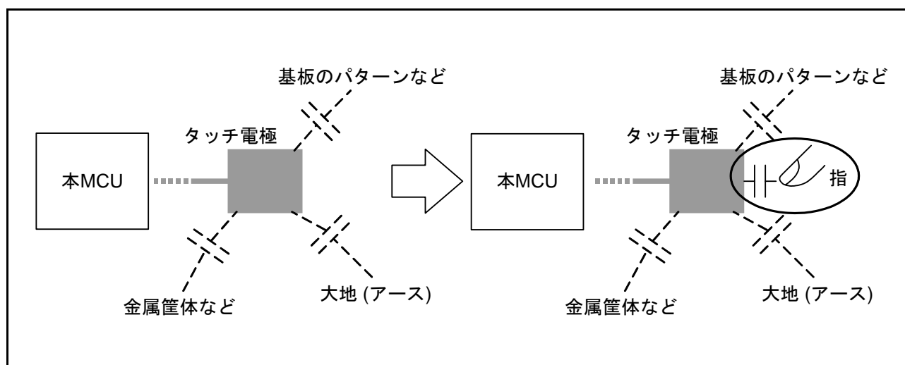
図 32.1 指による静電容量の増加
