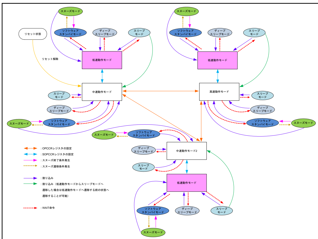
図 11.2 動作モード
