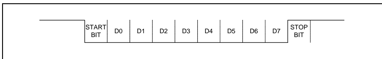
図 41.23 通信フォーマット
