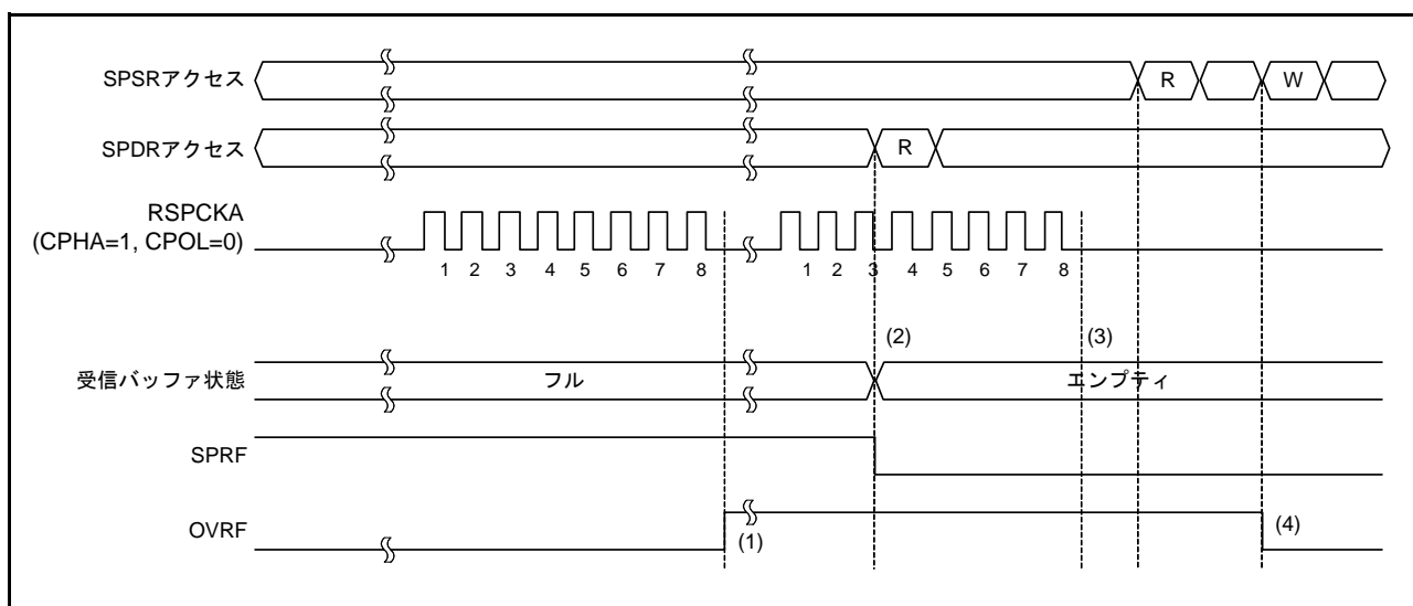
図 30.29 SPRF フラグと OVRF フラグの動作例
