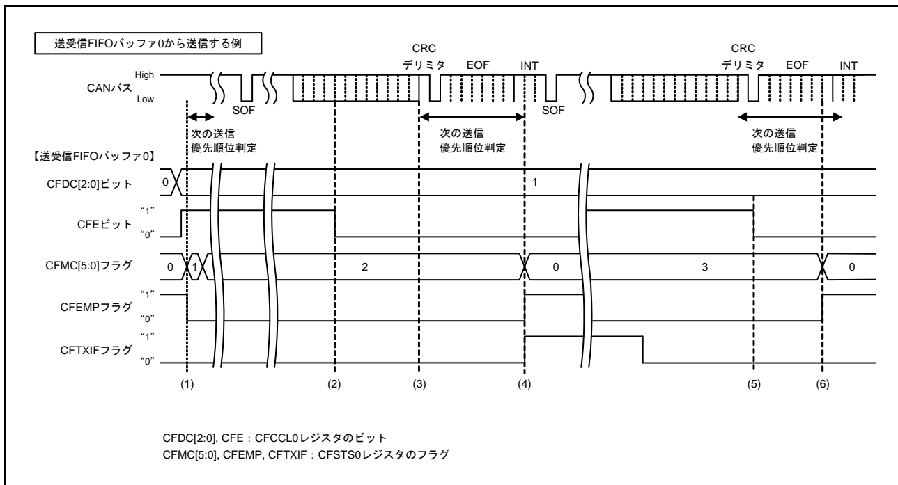
図 29.31 送受信 FIFO バッファの送信タイミング図 (送信アボート完了時)
