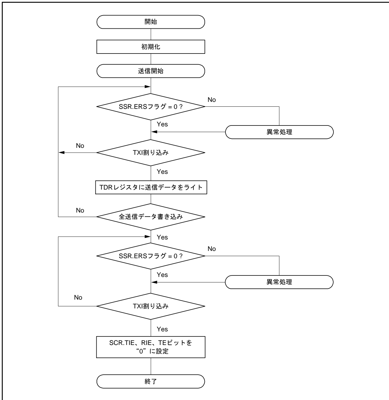
図 27.45 スマートカードインタフェース送信のフローチャート例
