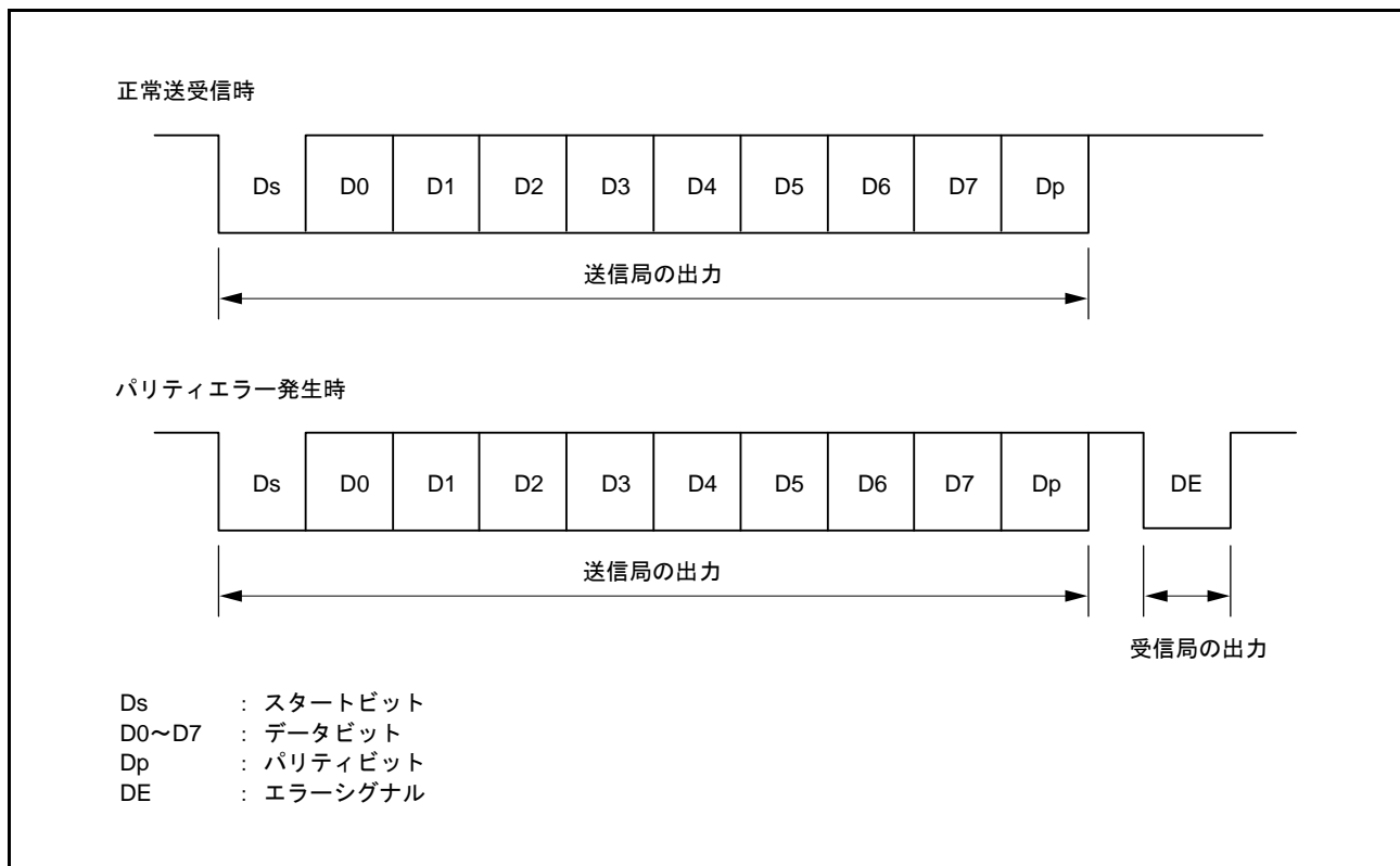
図 27.38 スマートカードインタフェースモードのデータフォーマット
