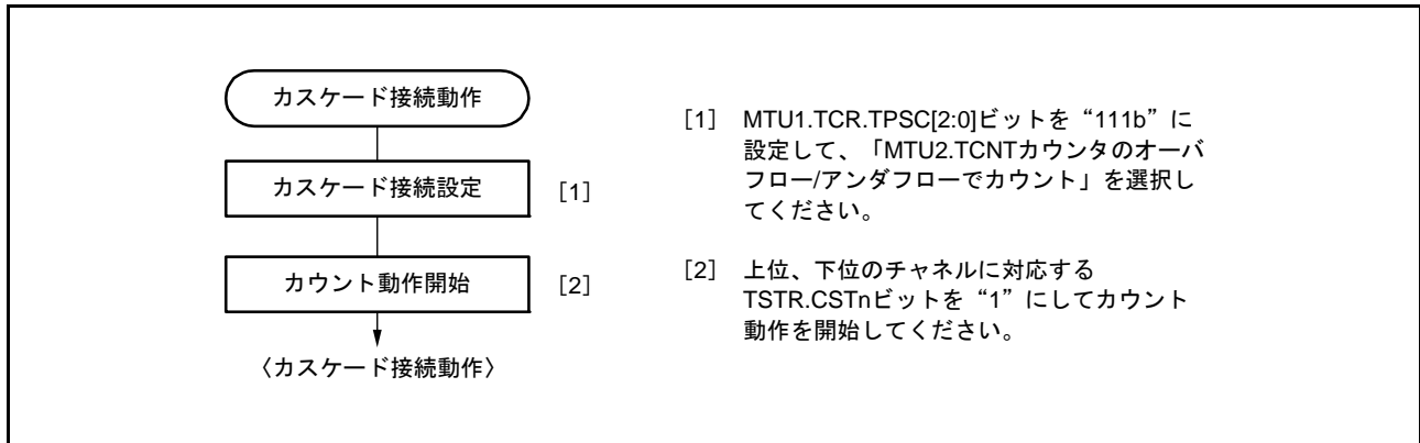
図 20.20 カスケード接続動作設定手順
