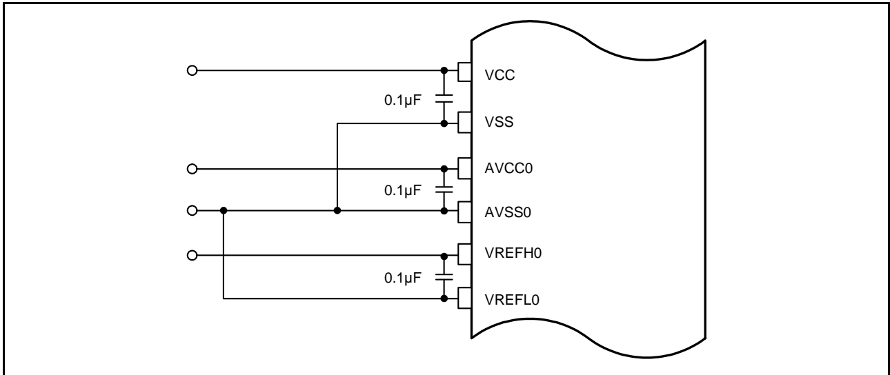
図 35.31 各電源端子の接続例
