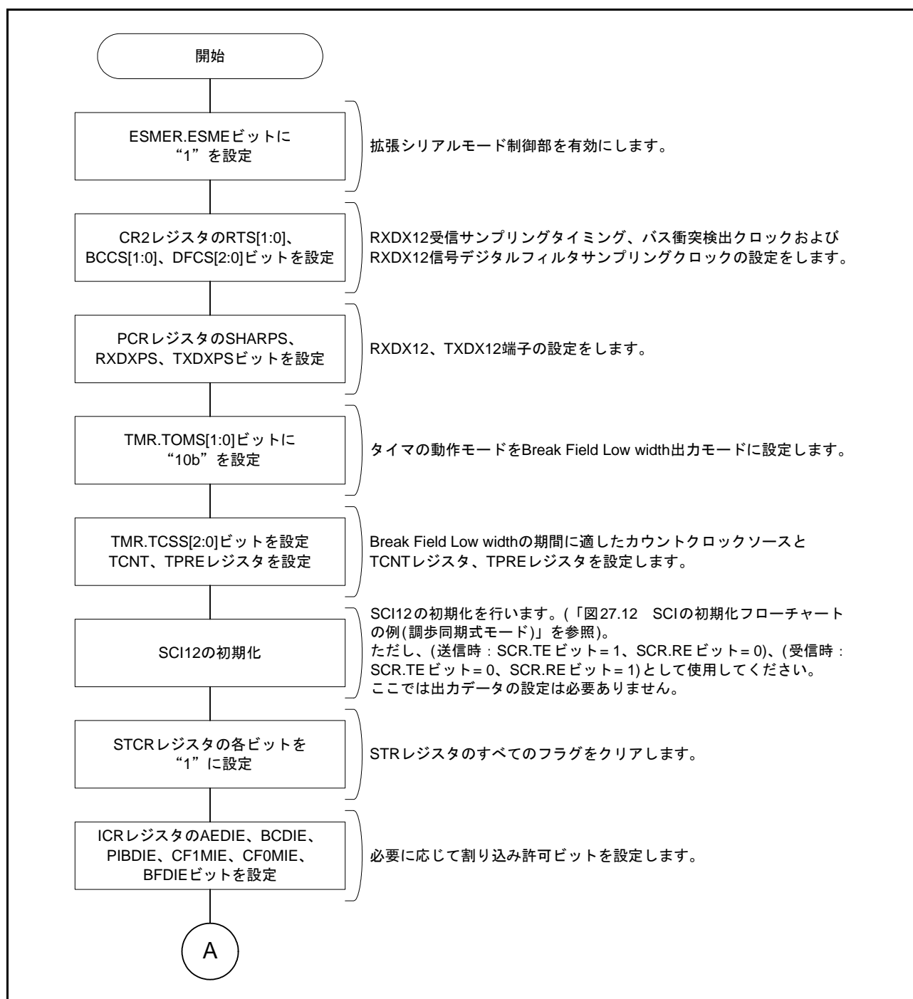
図 27.66 Start Frame 送信フローチャート例 (1)
