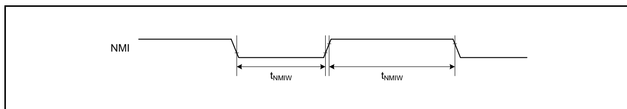
図 42.27 NMI 割り込み入力タイミング
