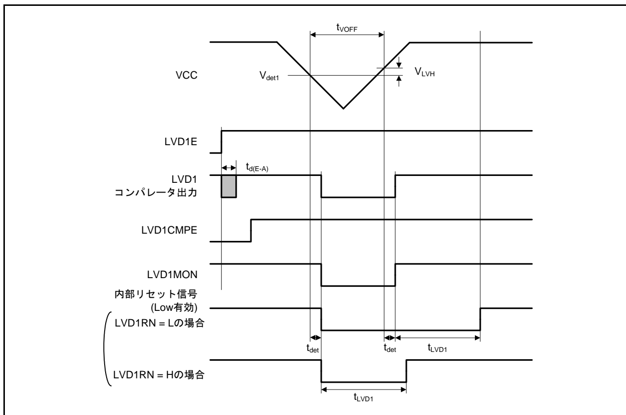
図 42.61 電圧検出回路タイミング ( V_{det1} )
