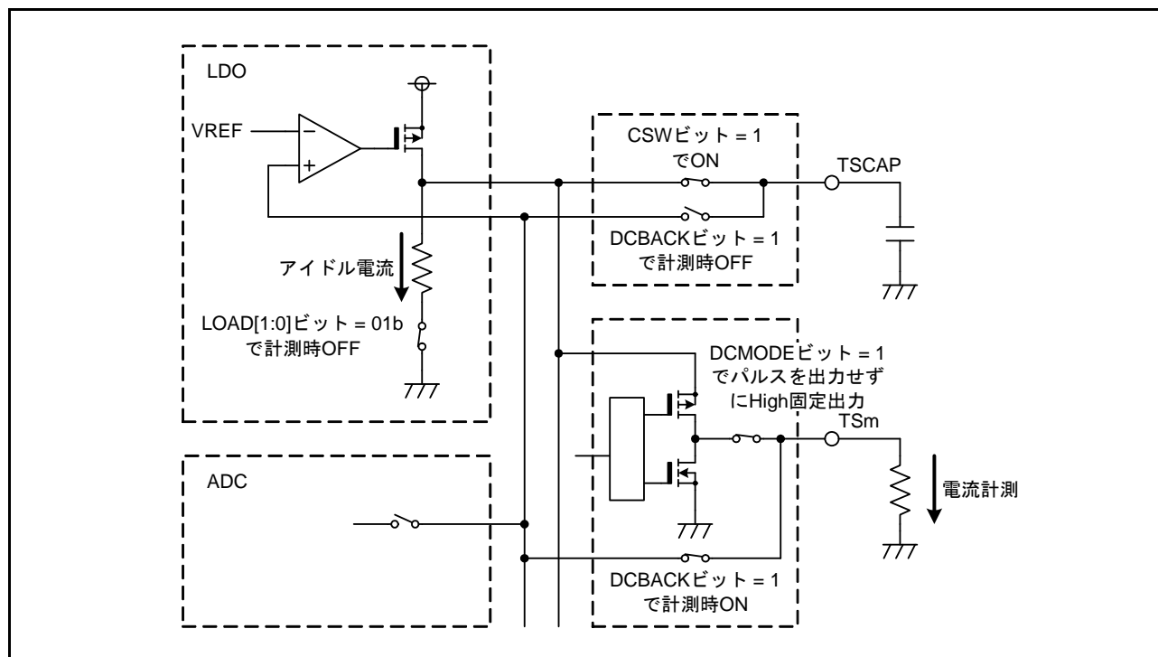
図 32.6 LDO のフィードバックループ
