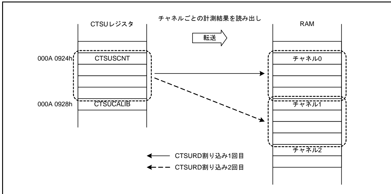
図 32.14 CTSURD 割り込みを用いた DTC 転送動作例
