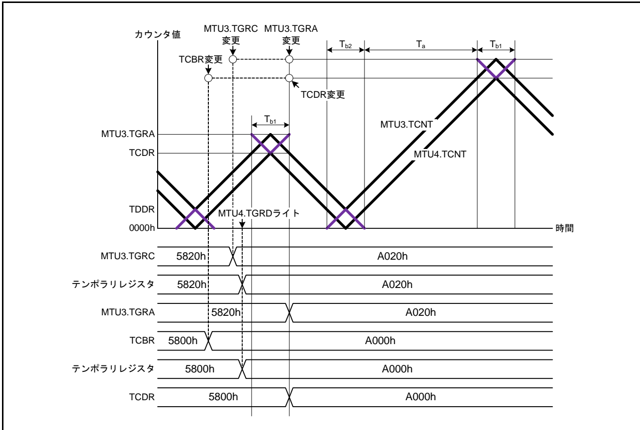
図 20.42 PWM 周期の変更例
