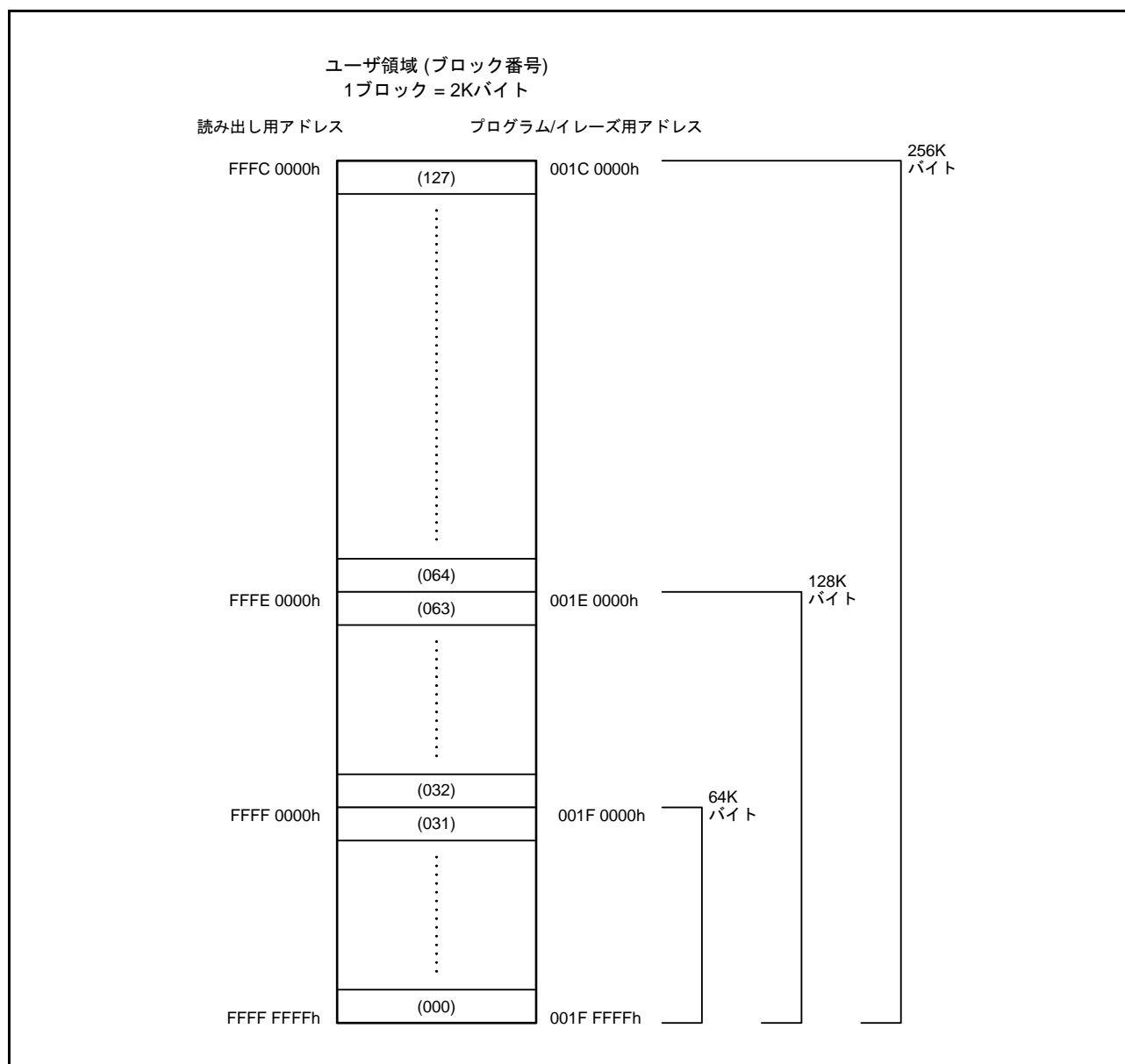
図 41.1 ROMの領域とブロックの構成
