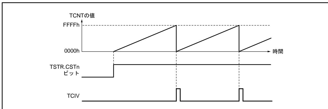
図 20.5 フリーランニングカウンタの動作
