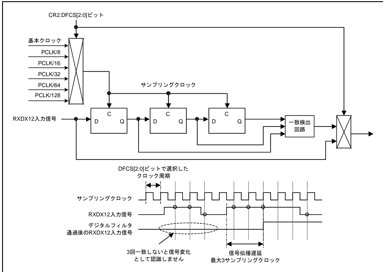
図 27.74 デジタルフィルタ機能の動作例
