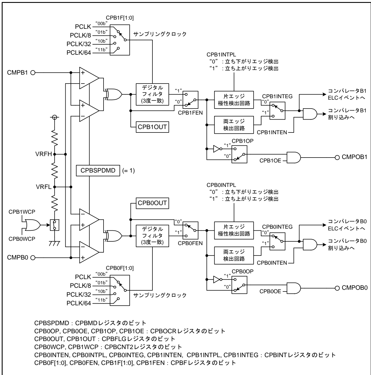
図 38.2 コンパレータ B0、B1 のブロック図 (ウィンドウ機能が有効時)
