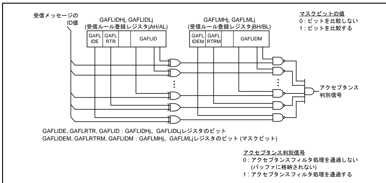
図 29.5 アクセプタンスフィルタ機能
