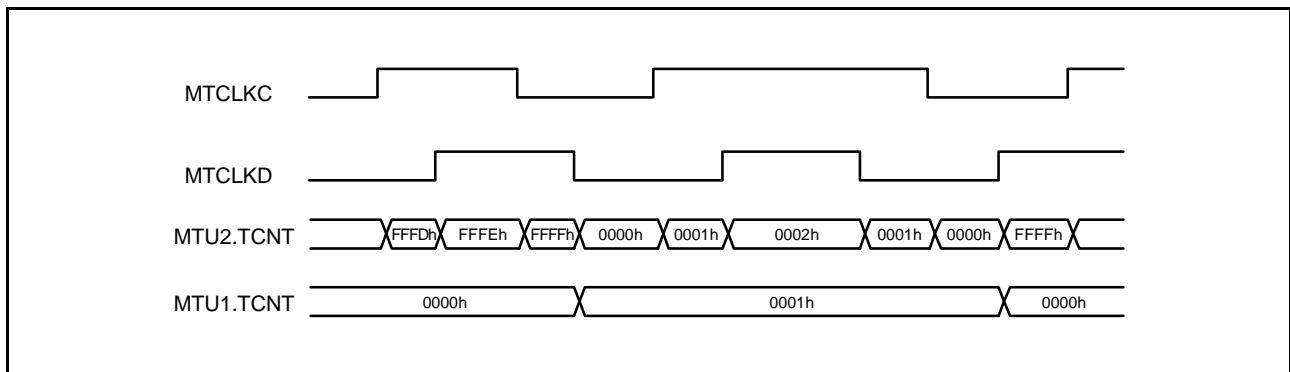
図 20.21 カスケード接続動作例 (a)
