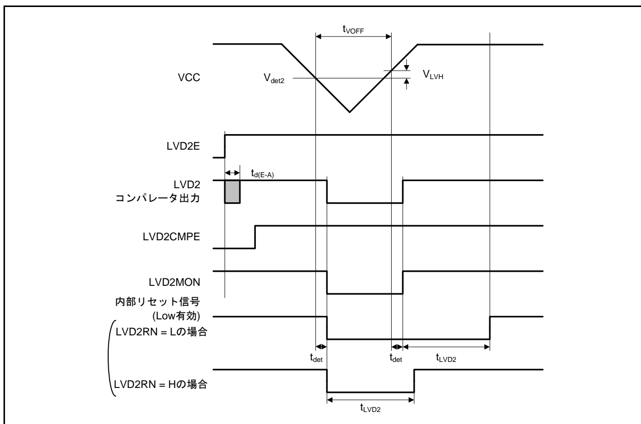
図 42.62 電圧検出回路タイミング ( V_{det2} )
