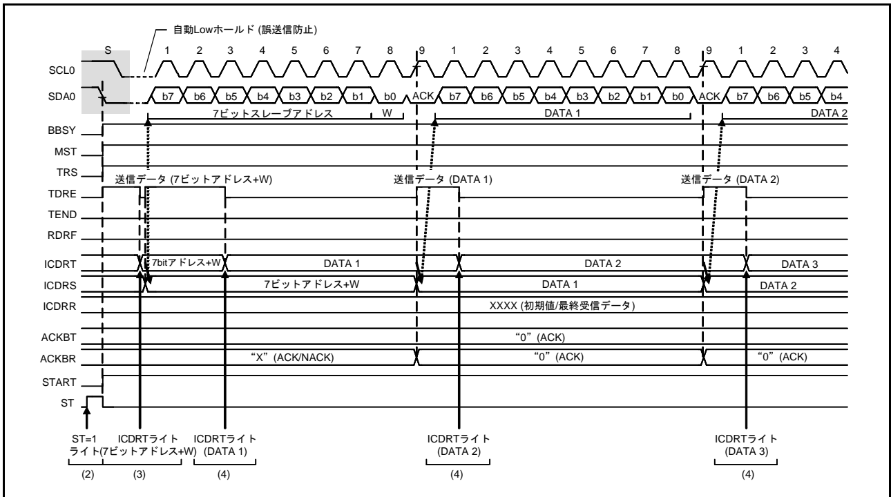
図 28.6 マスタ送信の動作タイミング (1) (7ビットアドレスフォーマットの時)
