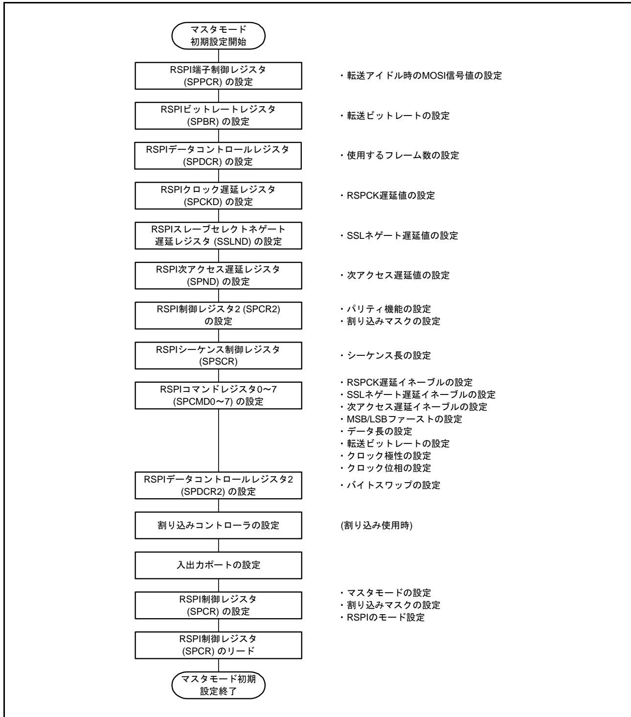
図 30.48 マスタモード時の初期化フロー例 (クロック同期式動作)
