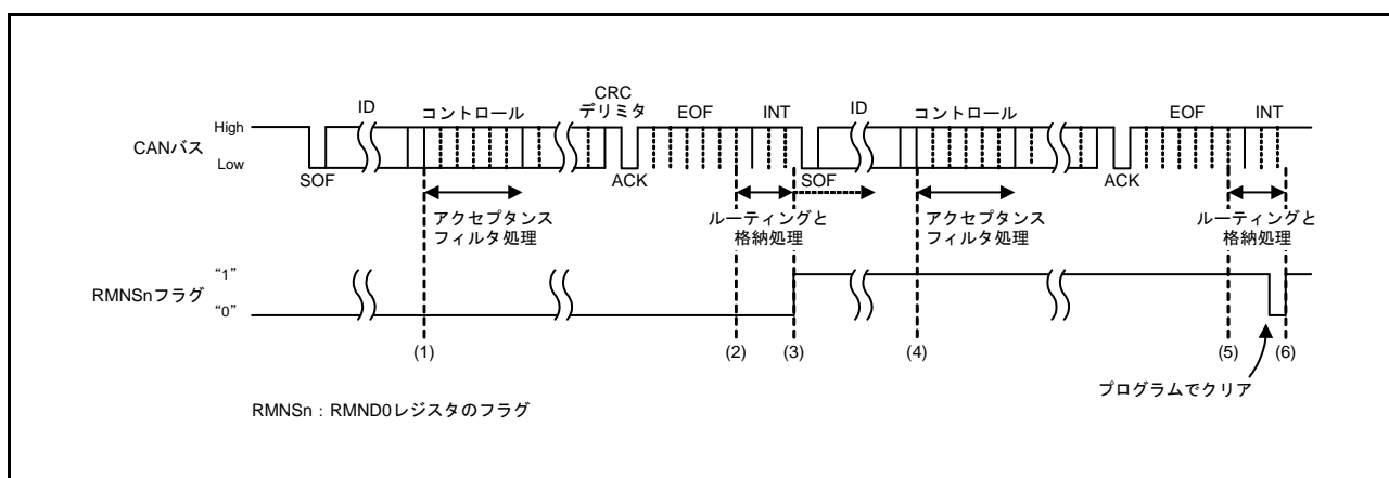
図 29.23 受信バッファの受信タイミング図
