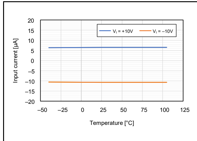
図 42.81 アナログ入力電流の温度依存性 ( AVCC0 = 5.0V 、 f_{MOD} = 4MHz 、総合 OSR = 4096 )
