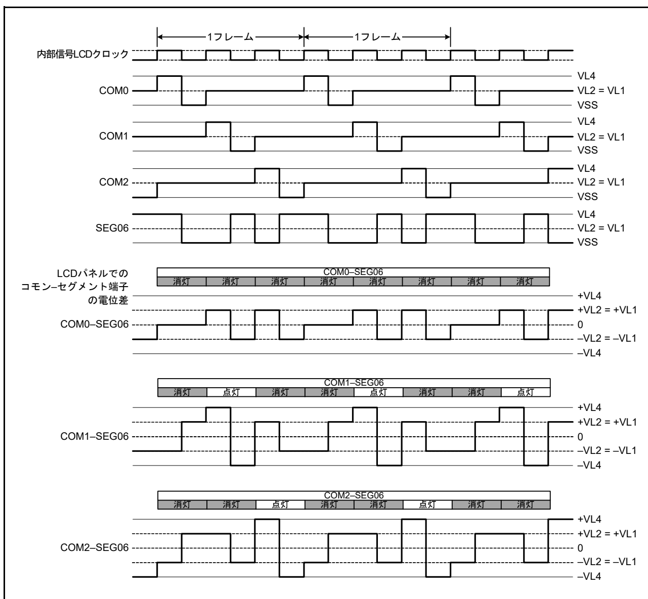
図 34.26 SEG06 端子と各コモン端子間の 1/3 デューティ LCD 駆動波形例 (1/2 バイアス)
