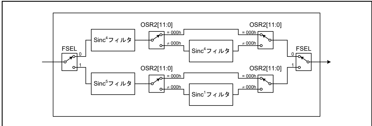
図 36.11 デジタルフィルタのブロック図
