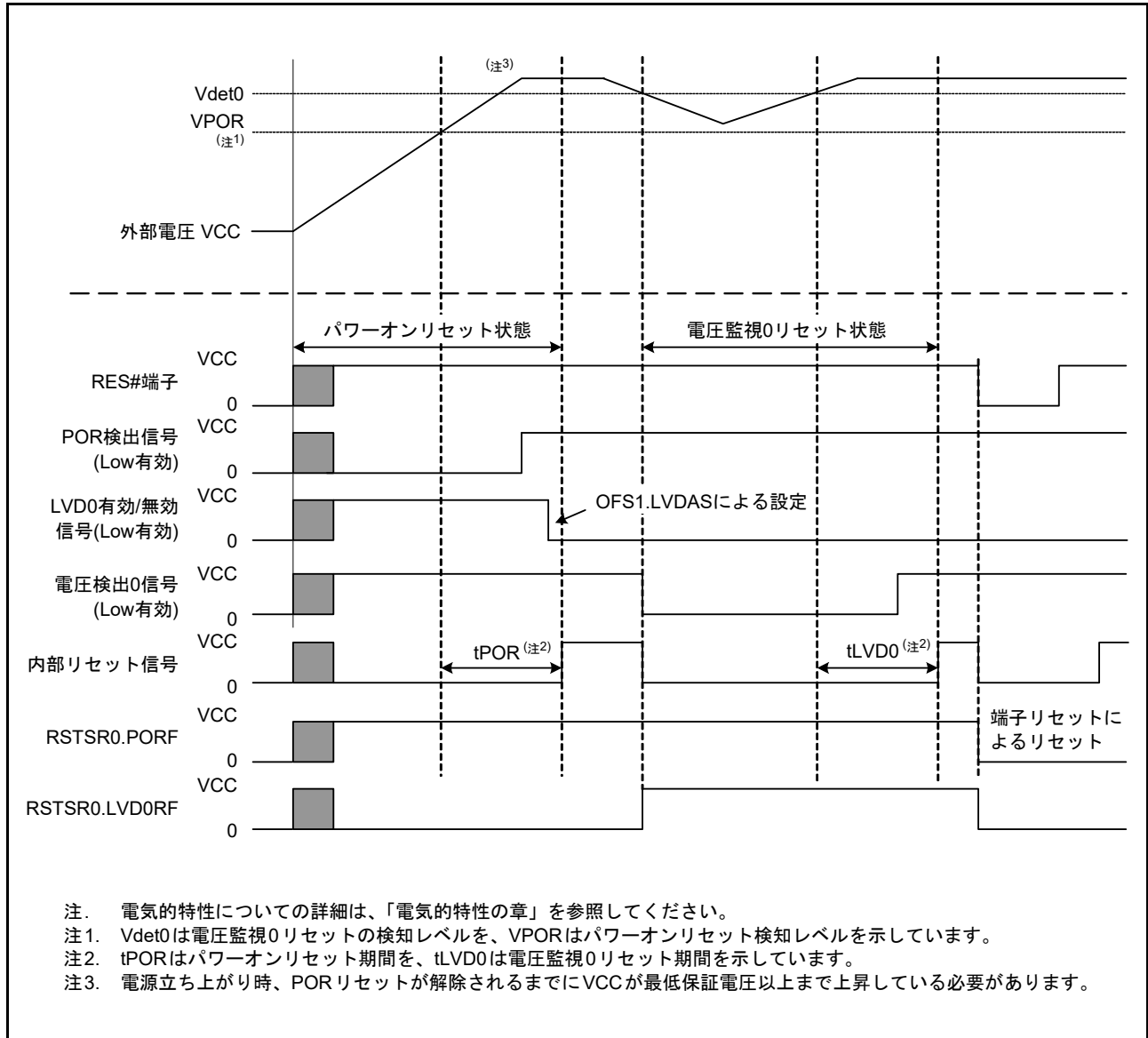
図 8.4 電圧監視 0 リセット動作例
