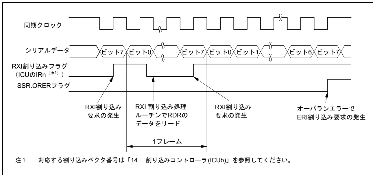
図 29.29 クロック同期式モードのシリアル受信時の動作例 (1) (RTS 機能未使用時)
