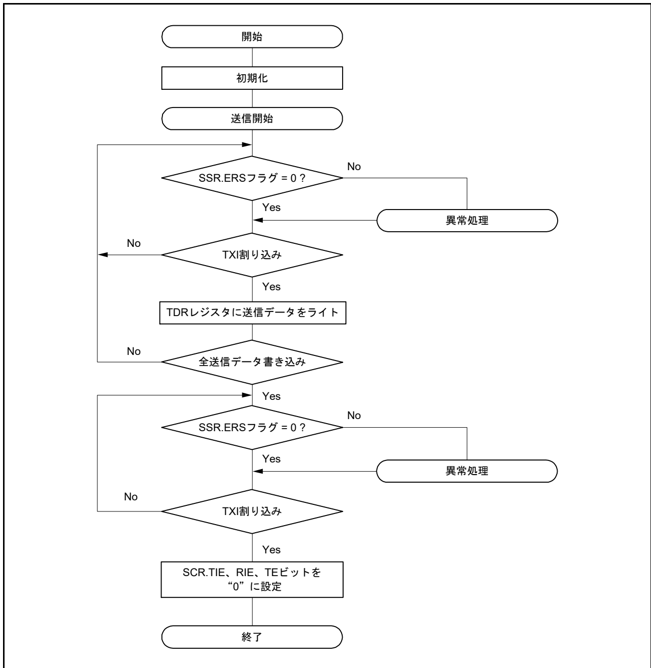
図 29.41 スマートカードインタフェース送信のフローチャート例
