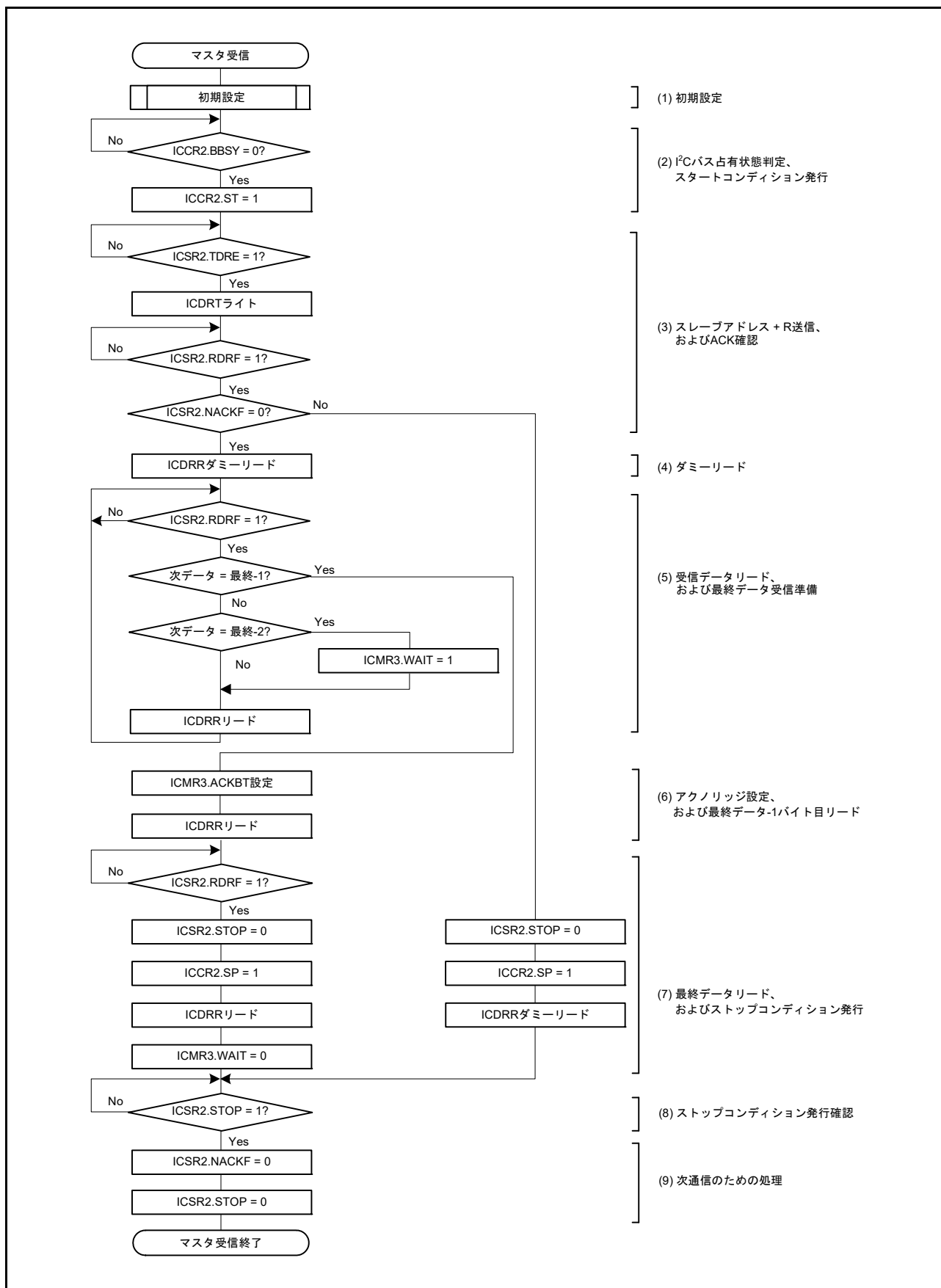
図 30.10 マスタ受信のフローチャート例 (7ビットアドレスフォーマット、3バイト以上の場合)
