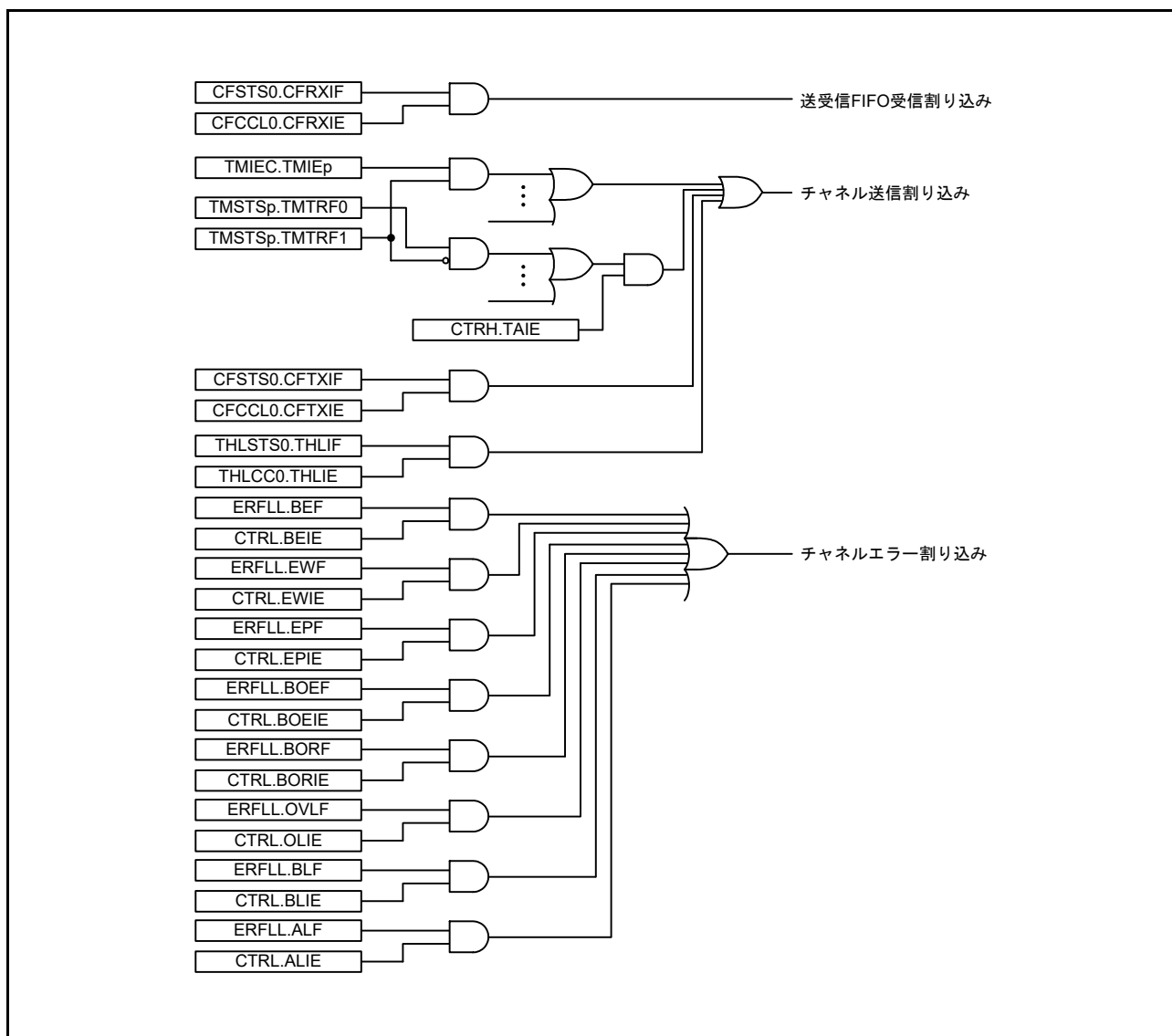
図 31.14 CAN チャンネル割り込みブロック図
