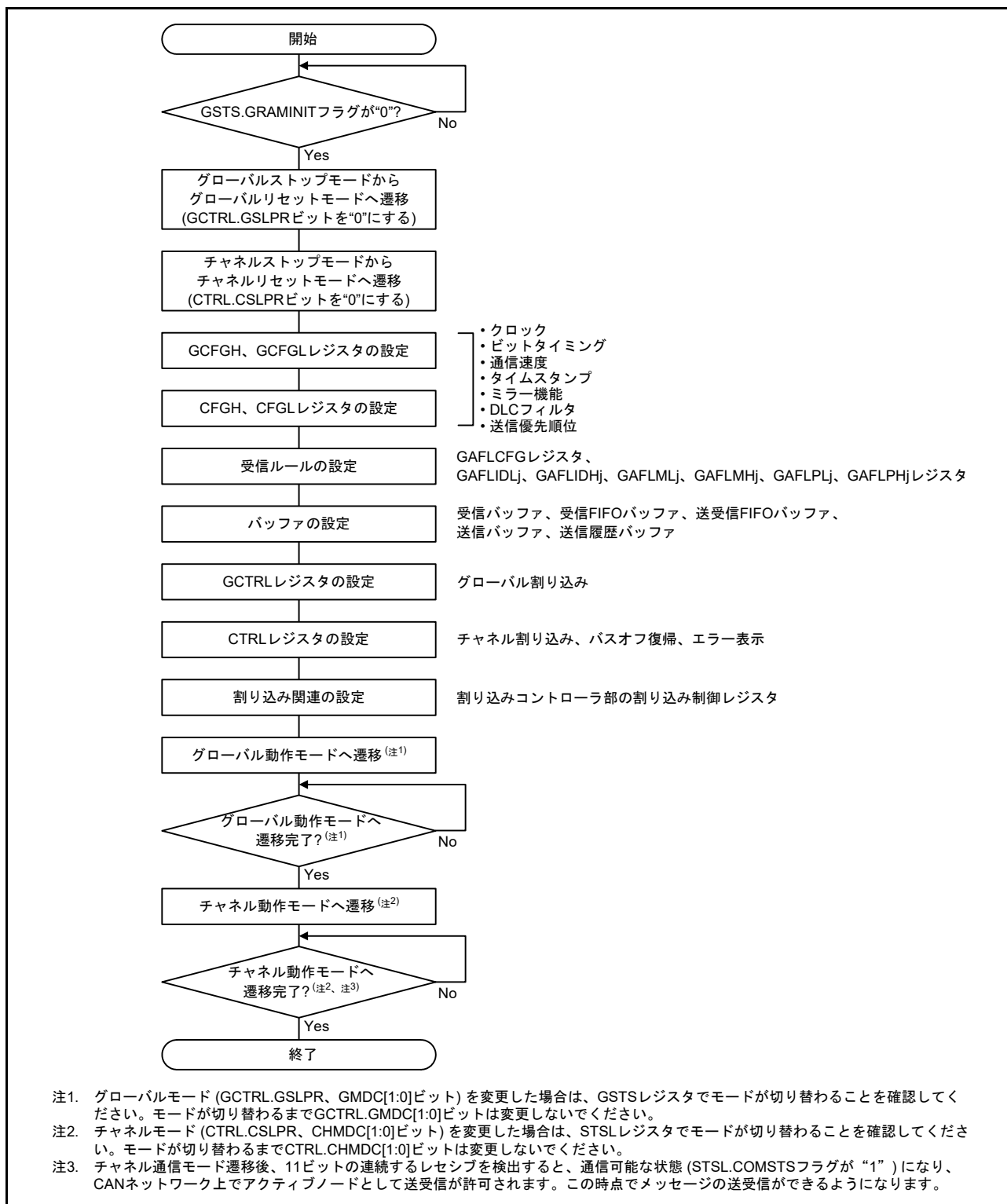
図 31.16 CAN モジュールイネーブル後の設定手順
