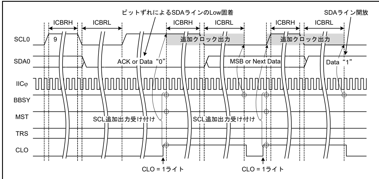
図 30.39 SCL 追加出力機能 (CLO ビット)
