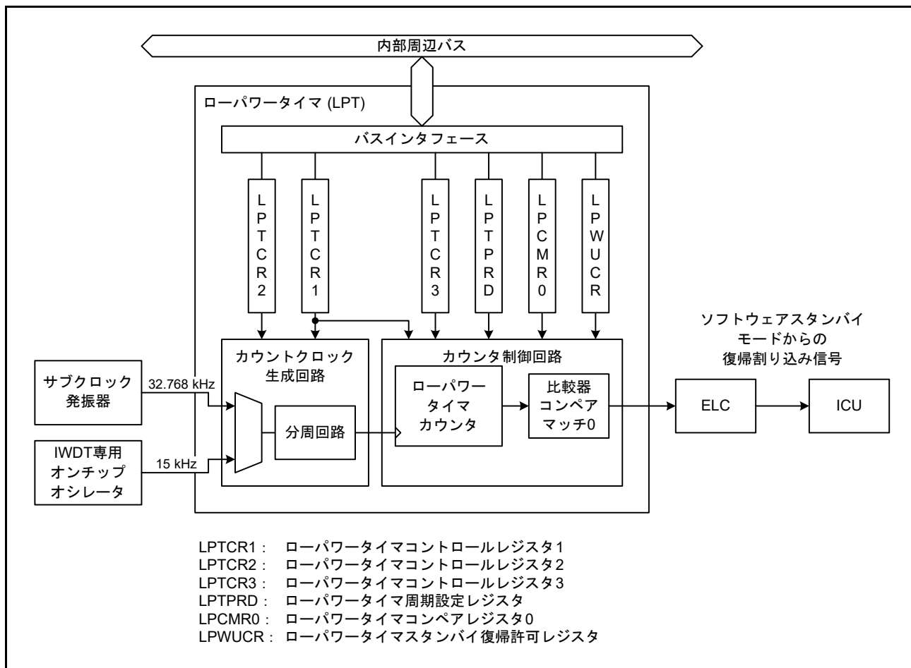
図 27.1 LPT のブロック図
