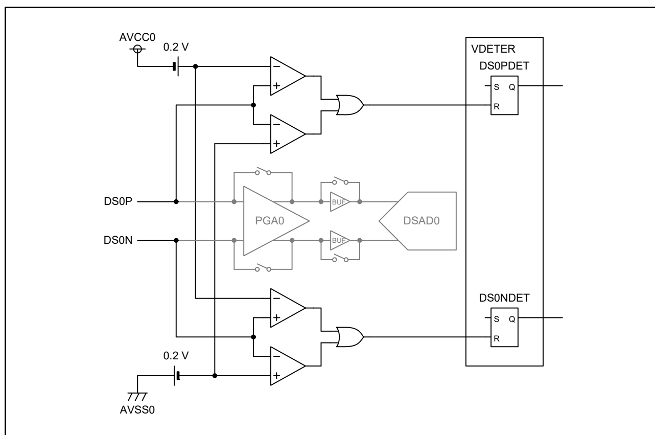
図 35.11 DSIDET のブロック図
