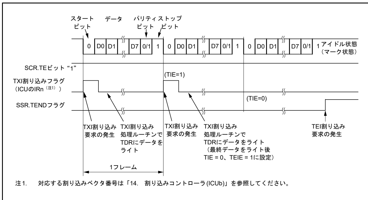
図 29.12 調歩同期式モードのシリアル送信の動作例 (3) (8ビットデータ / パリティあり / 1ストップビット / CTS機能使用しない / 送信中～送信終了時)
