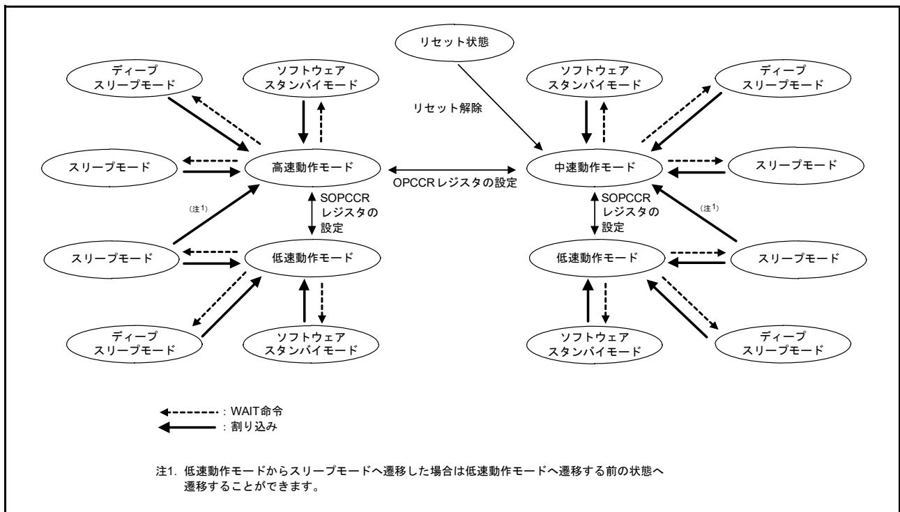
図 11.2 動作モード
