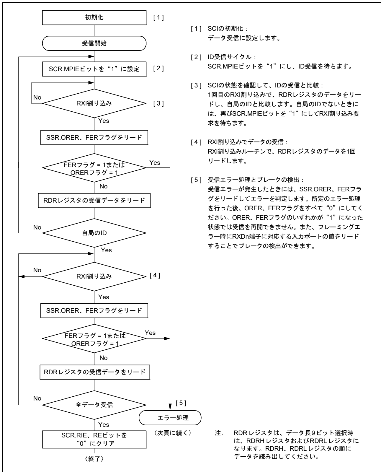
図 29.21 マルチプロセッサシリアル受信のフローチャートの例 (1)
