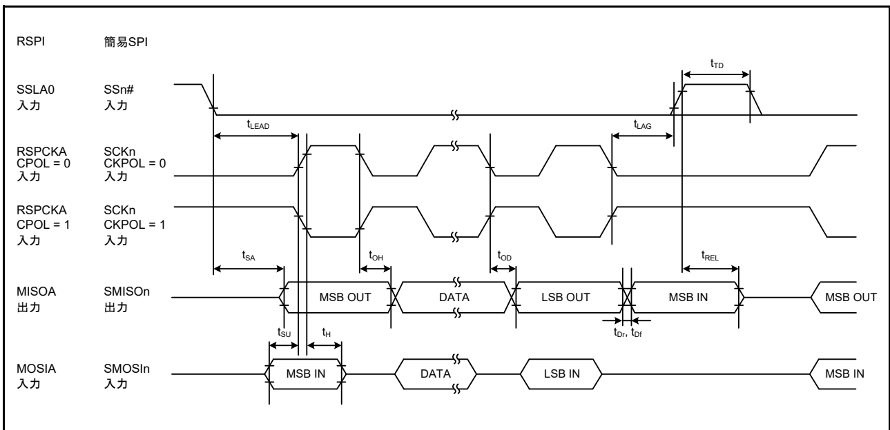
図 42.46 RSPCI タイミング (スレーブ、CPHA = 0)/ 簡易 SPI クロックタイミング (スレーブ、CKPH = 1) (n = 0, 1, 5, 6, 8, 9, 12)
