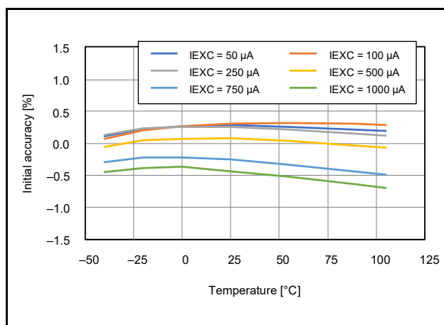
図 42.87 励起電流源出力電流の温度依存性 (AVCC0 = 5.0V)
