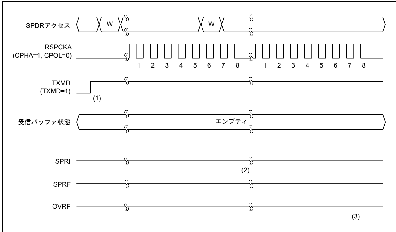
図 32.27 SPCR.TXMD = 1 の動作例
