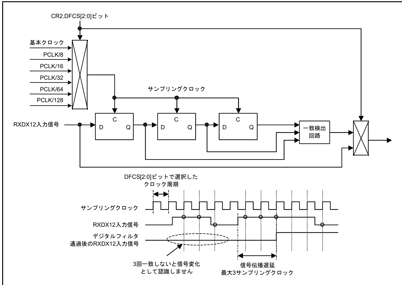
図 29.70 デジタルフィルタ機能の動作例
