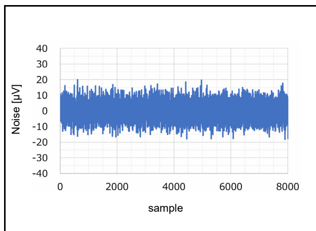
図 42.60 ノイズプロット (AVCC0 = 5.0V、 T_a = 25^\circ\text{C} 、Gain = 64、 f_{\text{MOD}} = 4\text{MHz} 、 f_{\text{DR}} = 125\text{k SPS} 、Sinc 5 フィルタ、 V_{\text{ID}} = 0\text{V} 、 V_{\text{REF}} = 2.5\text{V} 、リファレンスバッファ無効)
