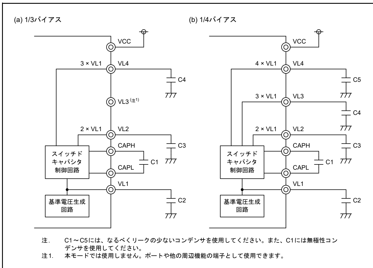
図 34.11 LCD バイアス電圧生成回路の外付け回路例 (内部昇圧方式)
