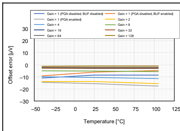
図 42.70 オフセット誤差の温度依存性 (AVCC0 = 5.0V、 V_{\text{ID}} = 0\text{V} 、 f_{\text{MOD}} = 4\text{MHz} 、総合 OSR = 4096、 V_{\text{REF}} = 2.5\text{V} )
