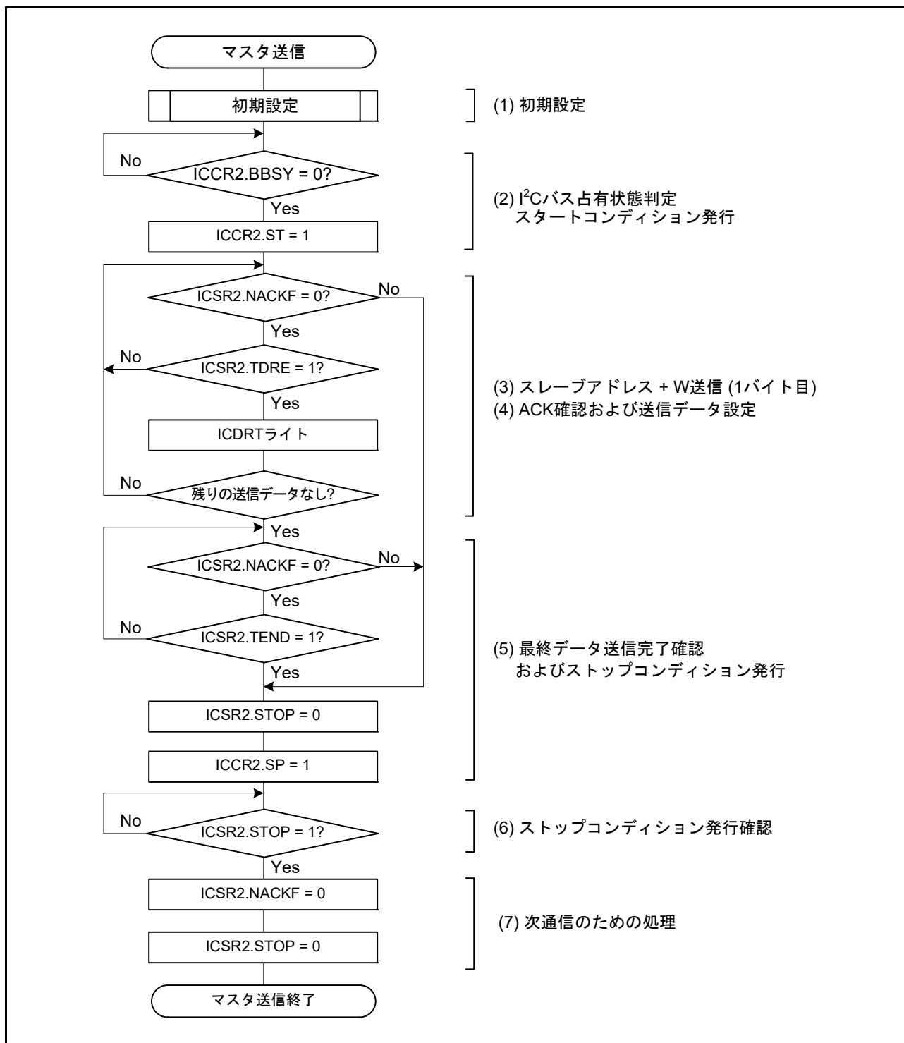
図 30.5 マスタ送信のフローチャート例
