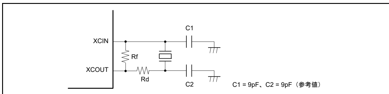
図 9.5 32.768kHz 水晶振動子の接続例
