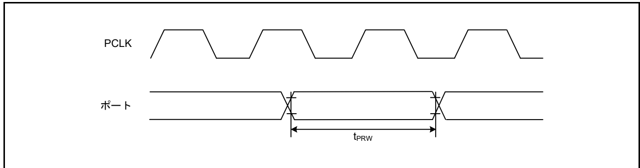
図 42.31 I/Oポート入力タイミング
