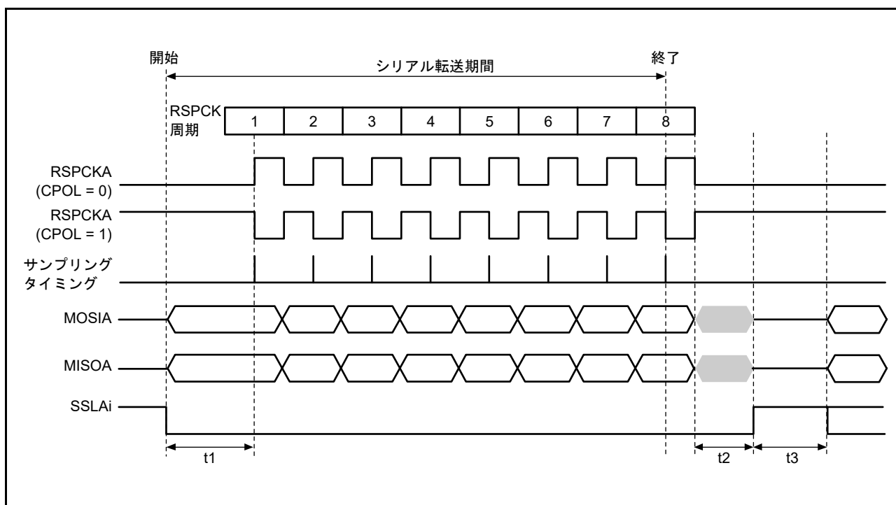
図 32.24 RSPI 転送フォーマット (CPHA ビット = 0)
