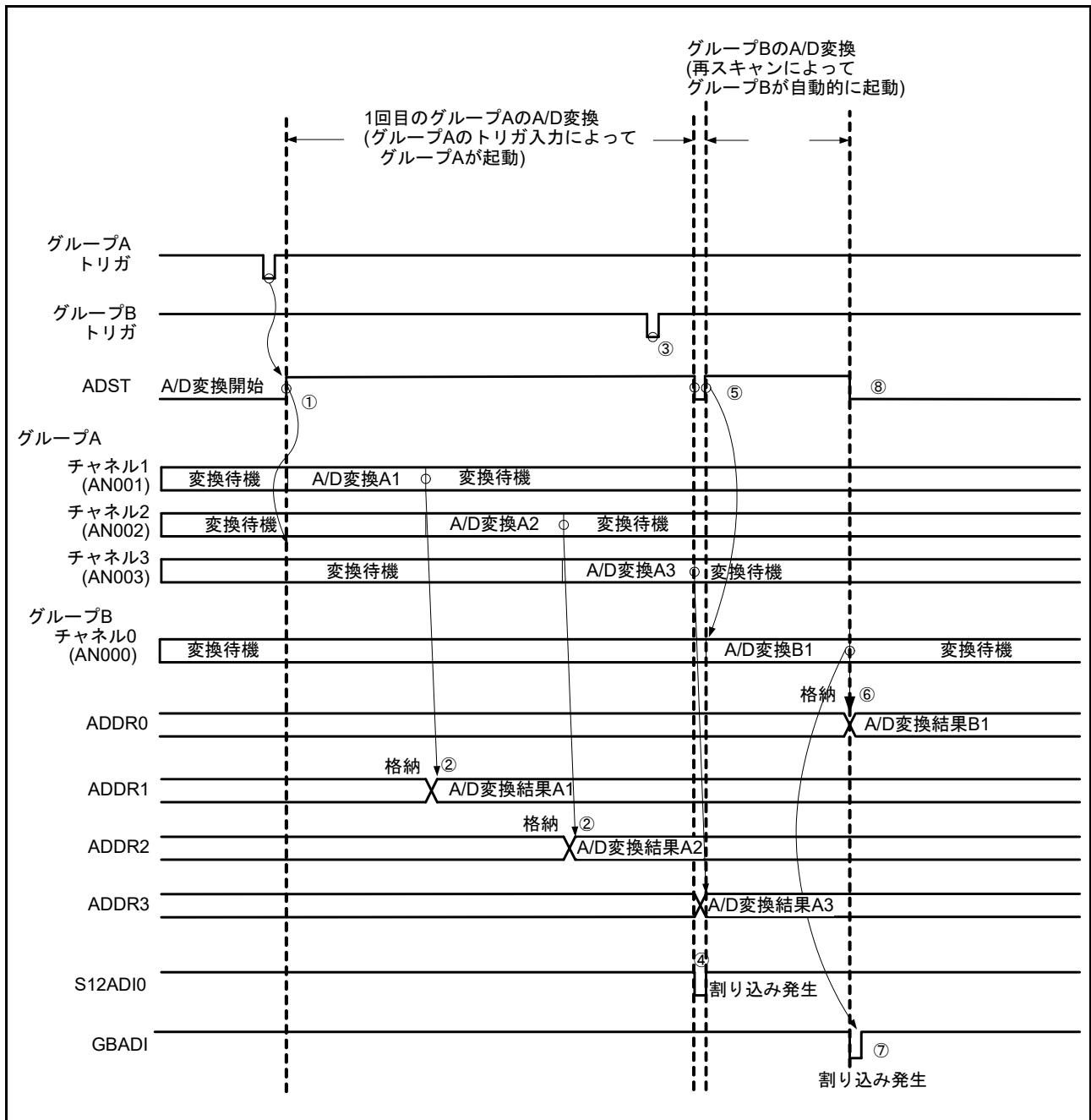
図 37.15 グループ A 優先制御の動作例 (3) (ADGSPCR.GBRSCN = 1、ADGSPCR.GBRP = 0 時の動作)
