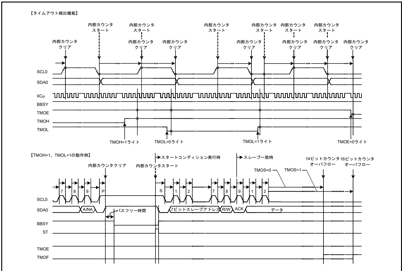
図 30.38 タイムアウト検出機能
