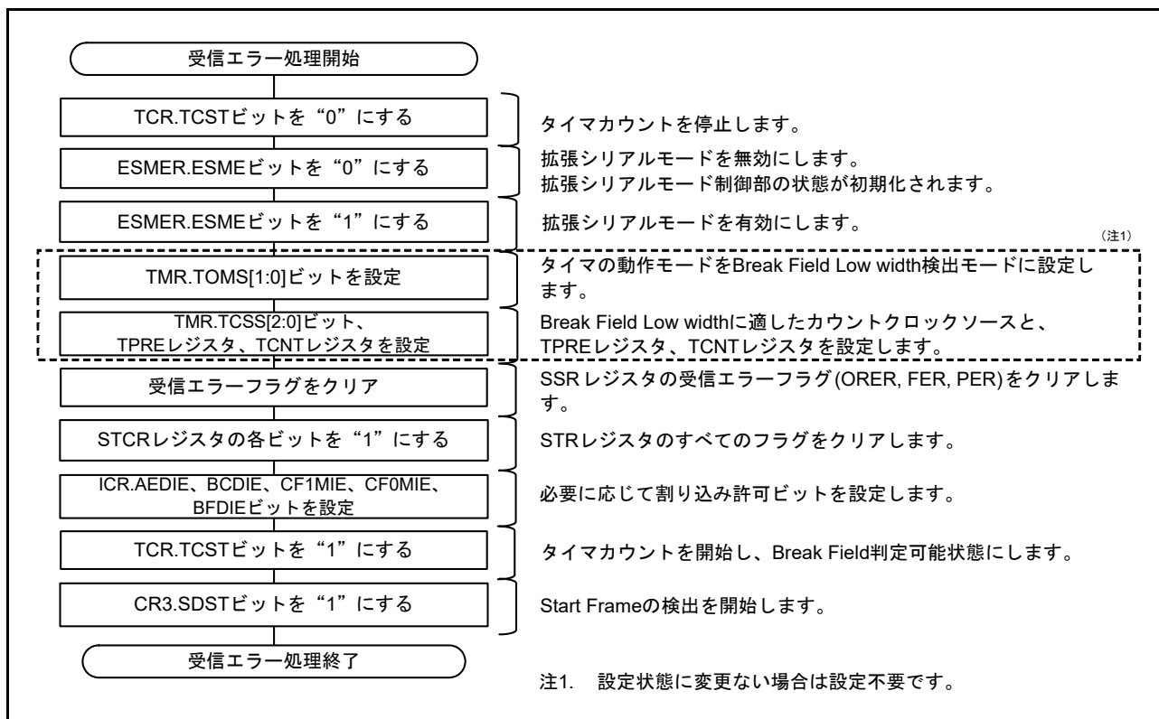
図 29.82 受信エラー処理のフローチャートの例 (Start Frame 受信中)
