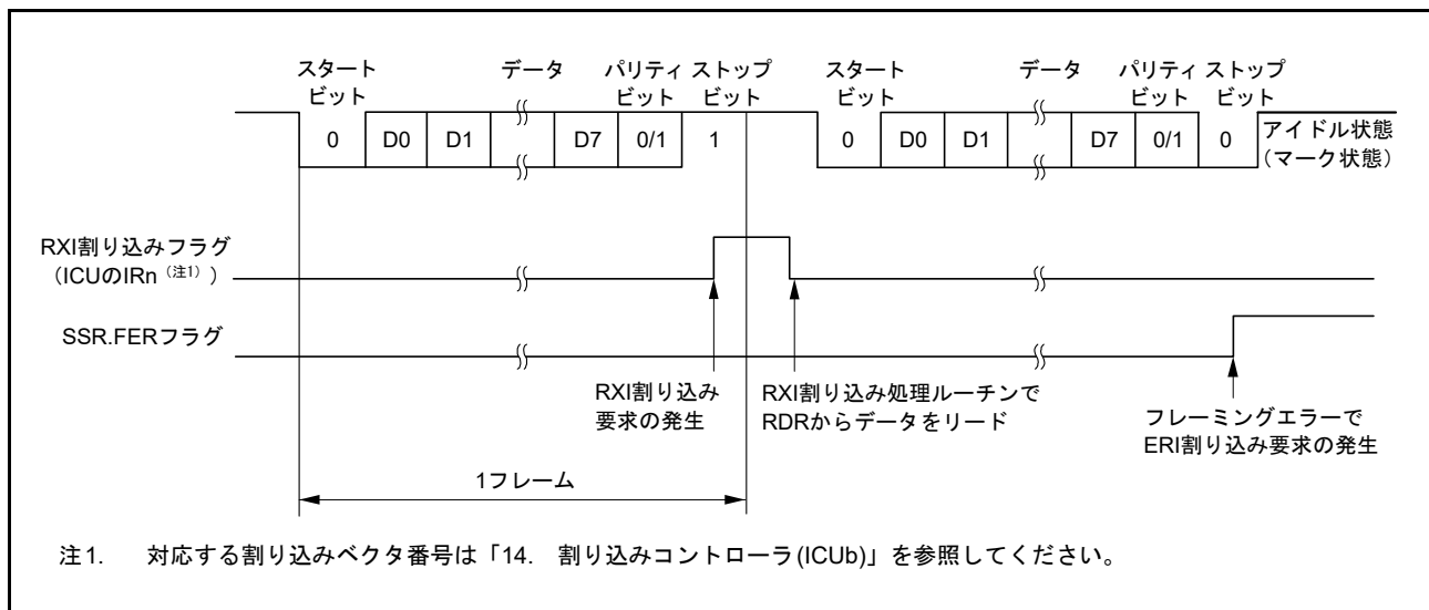
図 29.14 調歩同期式モードのシリアル受信時の動作例 (1) (RTS 機能未使用時) (8 ビットデータ / パリティあり / 1 ストップビットの例)
