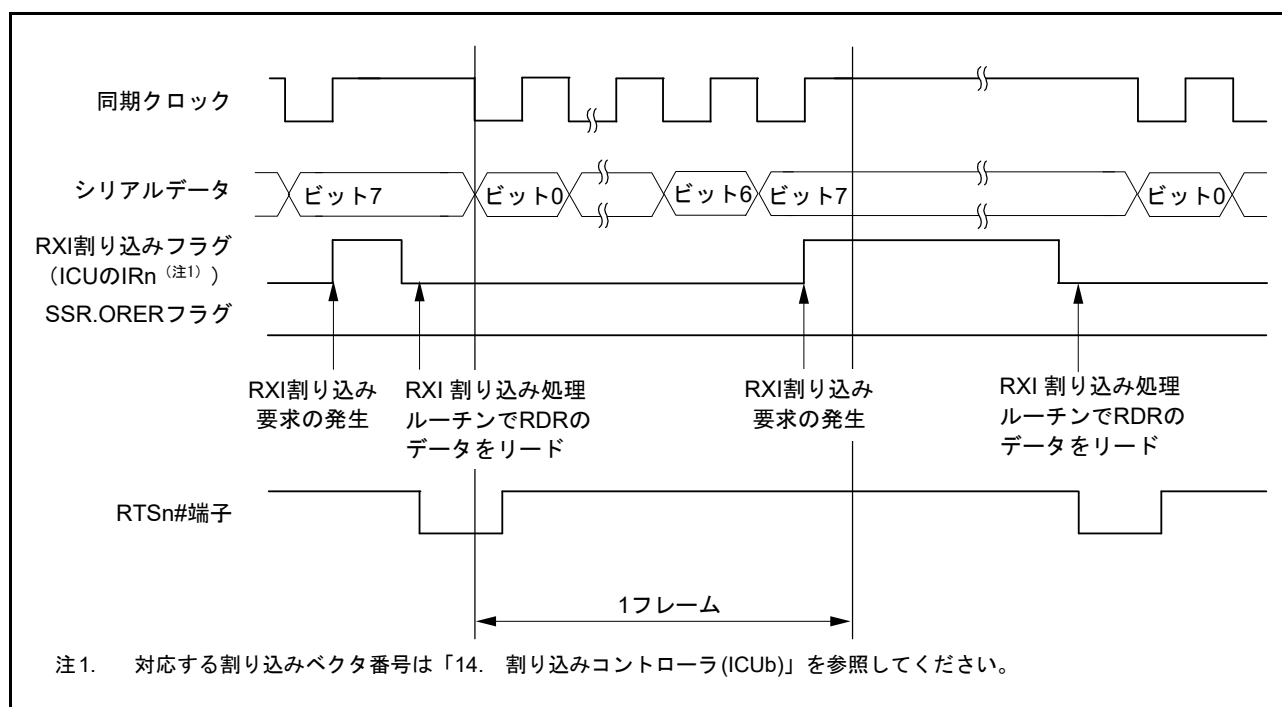
図 29.30 クロック同期式モードのシリアル受信時の動作例 (2) (RTS 機能使用時)
