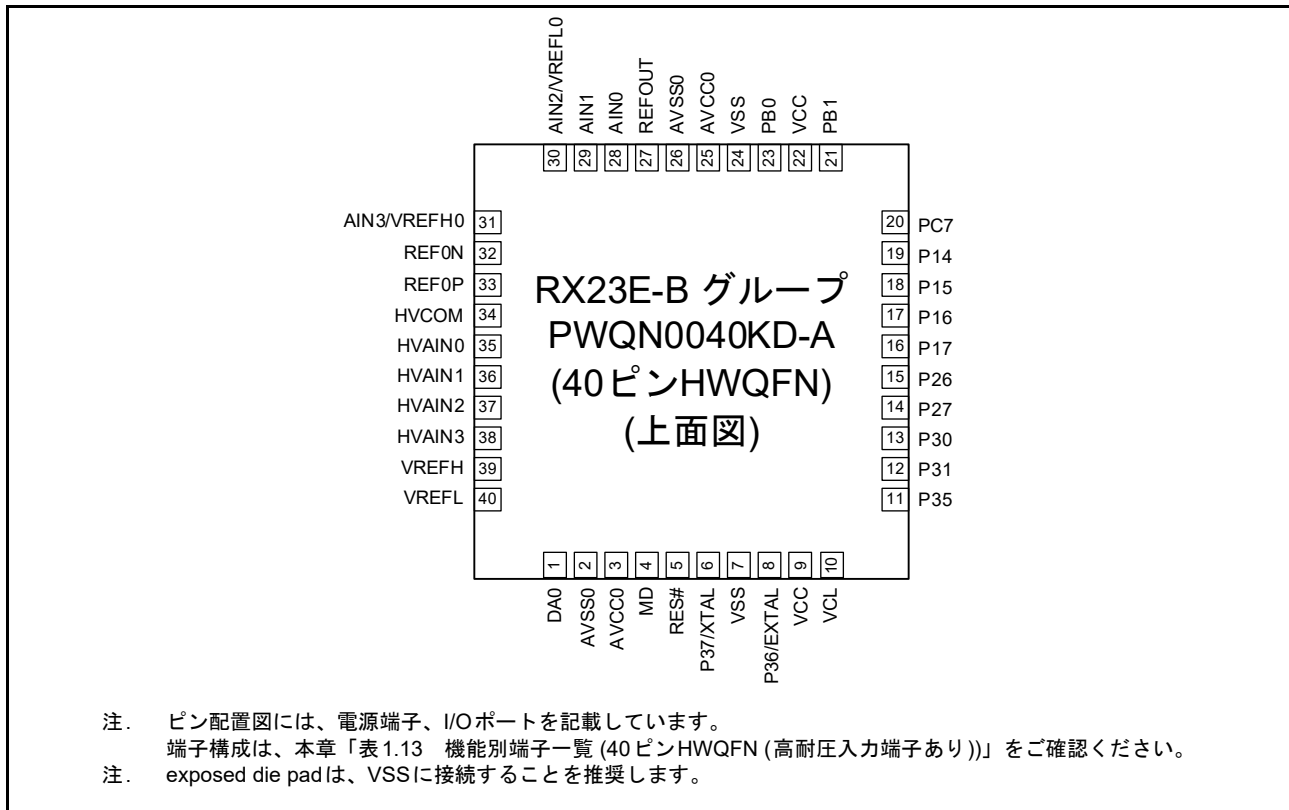
図 1.11 ピン配置図 (40ピン HWQFN (高耐圧入力端子あり))
