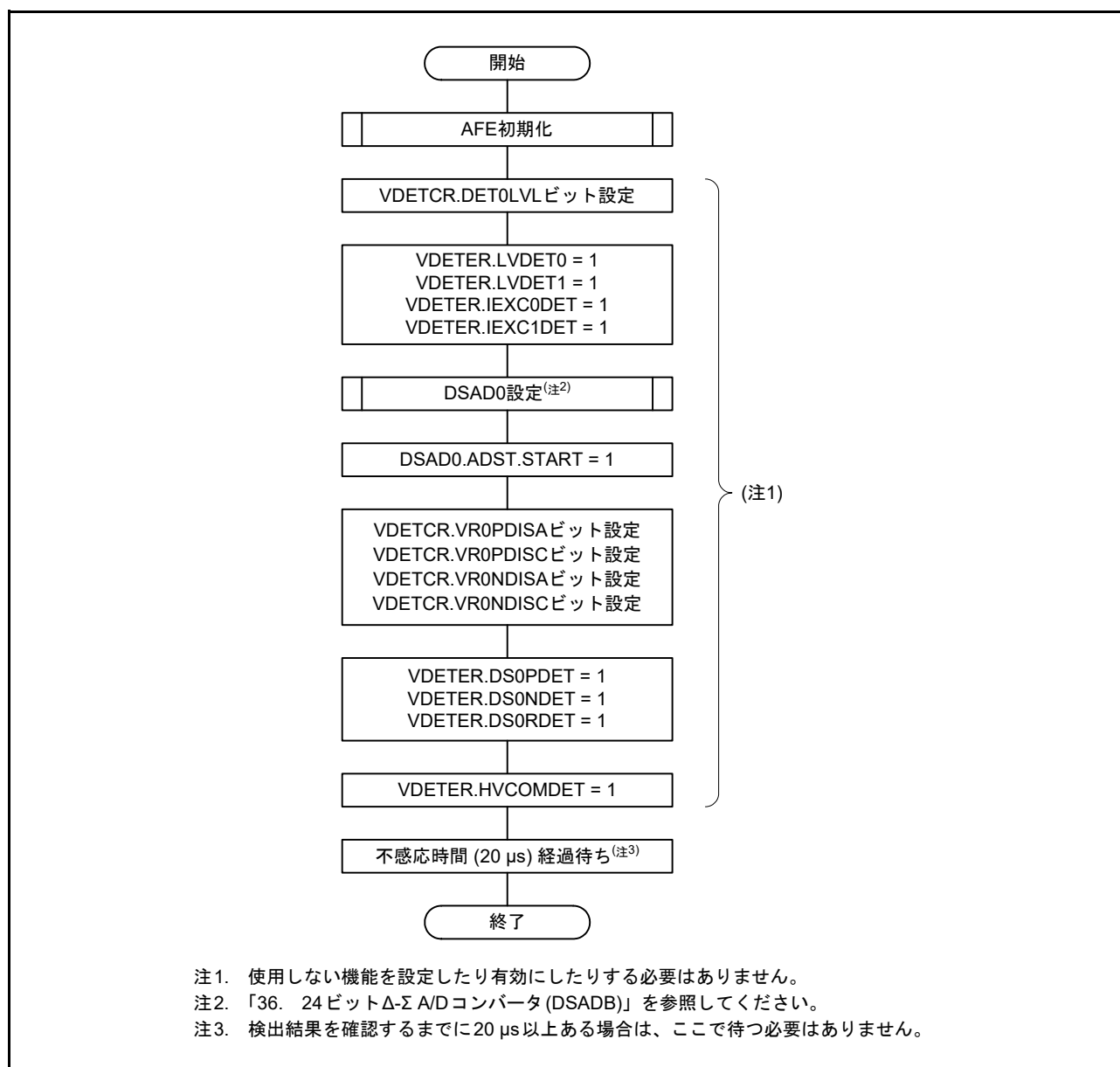
図 35.16 VDET の起動フロー
