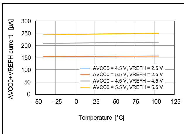
図 42.15 16 ビット D/A コンバータ動作電流の温度依存性
