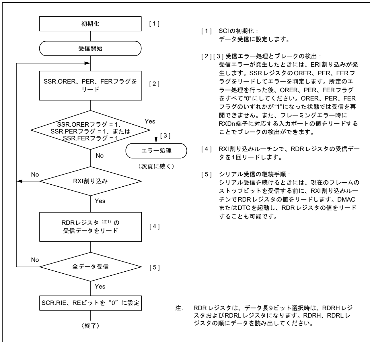
図 29.16 調歩同期式モードのシリアル受信のフローチャート例 (1)
