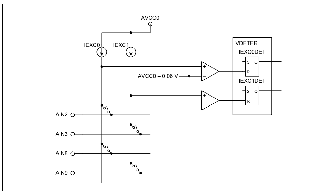
図 35.13 IEXCDET のブロック図
