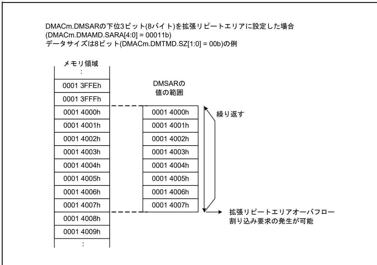
図 17.5 拡張リピートエリア機能の例
