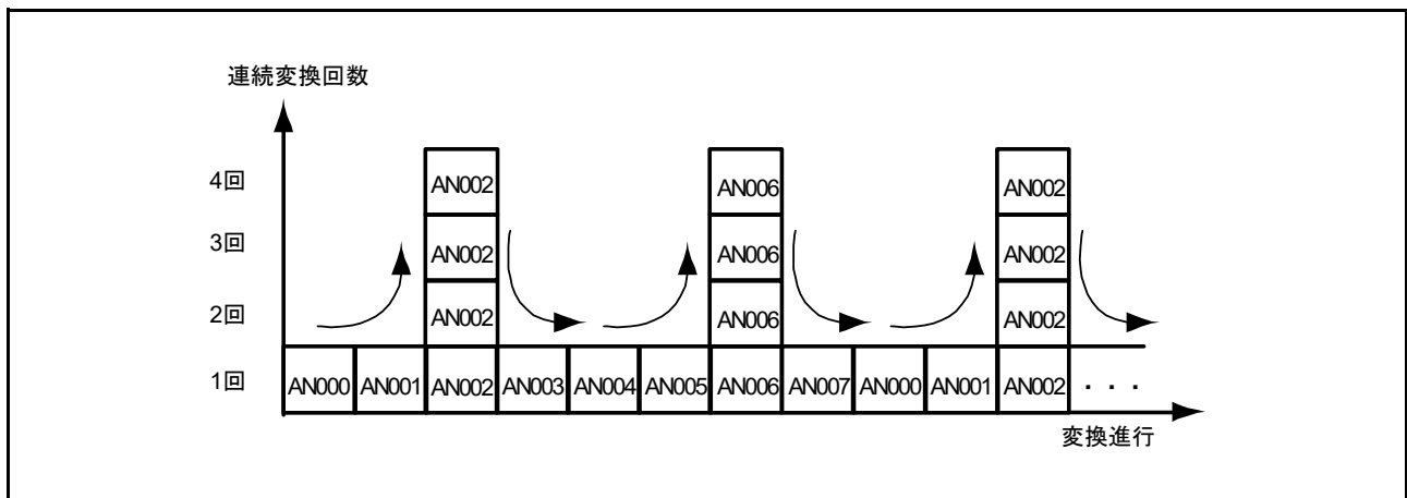
図 37.2 ADADC.ADC[2:0] = 011b、ADS002 = 1、ADS006 = 1 選択時のスキャン変換シーケンス
