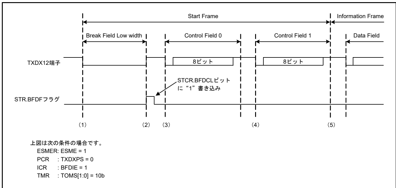
図 29.61 Start Frame 送信時の動作例
