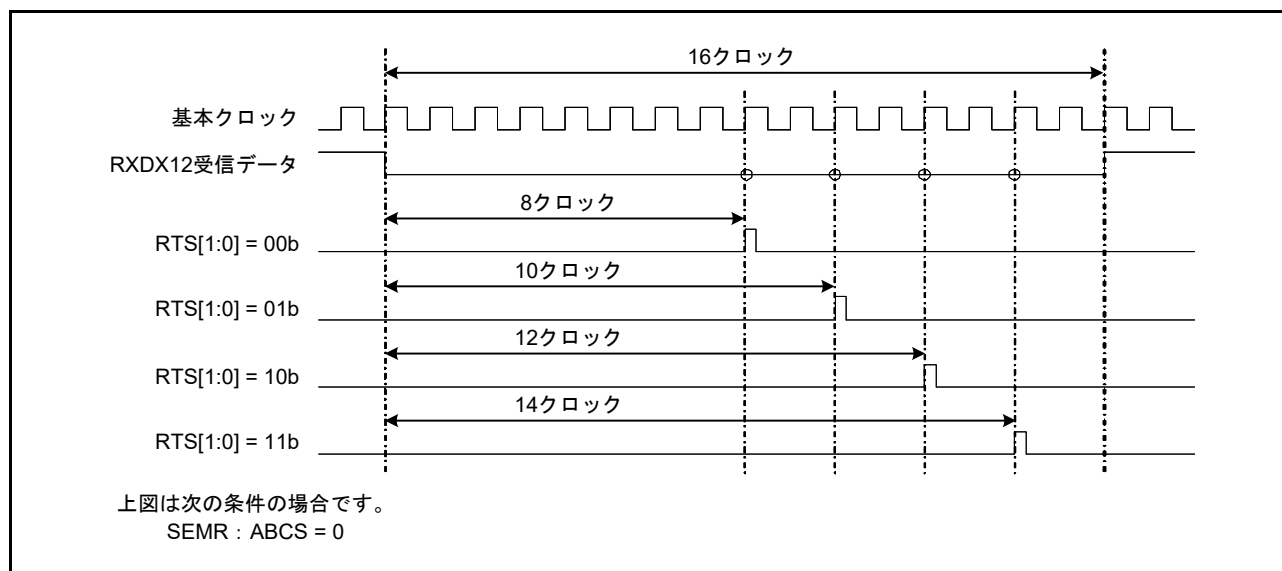
図 29.72 RXDX12 受信データサンプリングタイミング
