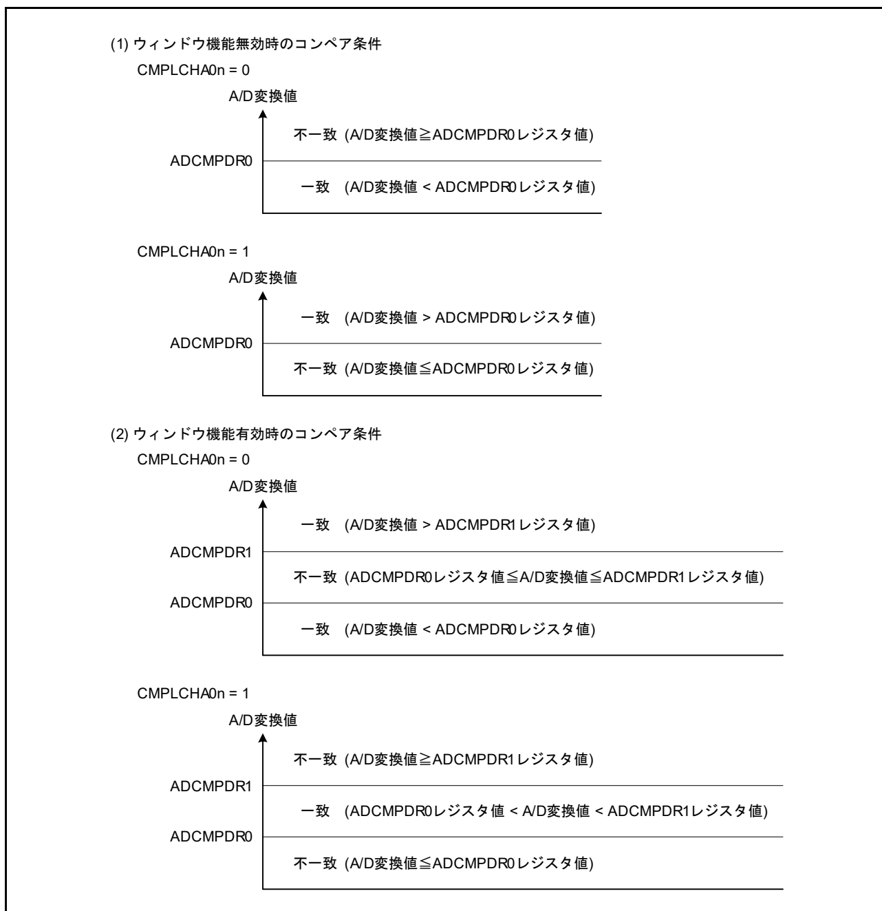
図 37.3 コンペア機能ウィンドウ A コンペア条件説明
