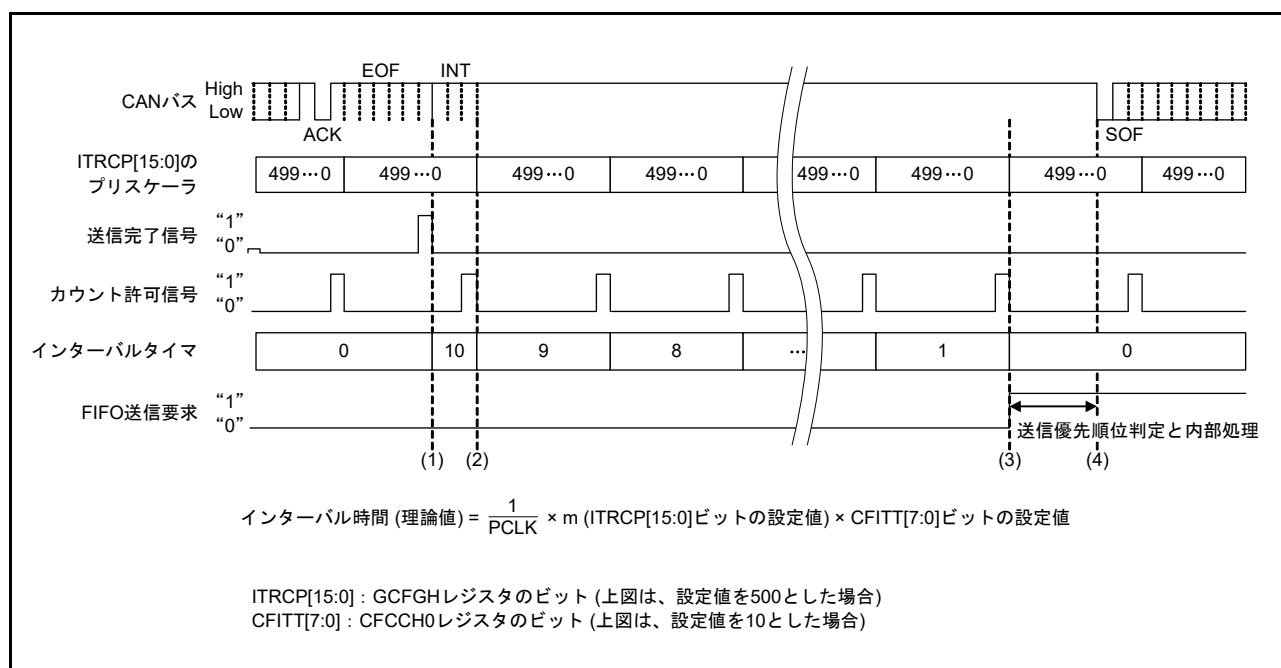
図 31.9 インターバルタイマのタイミング図
