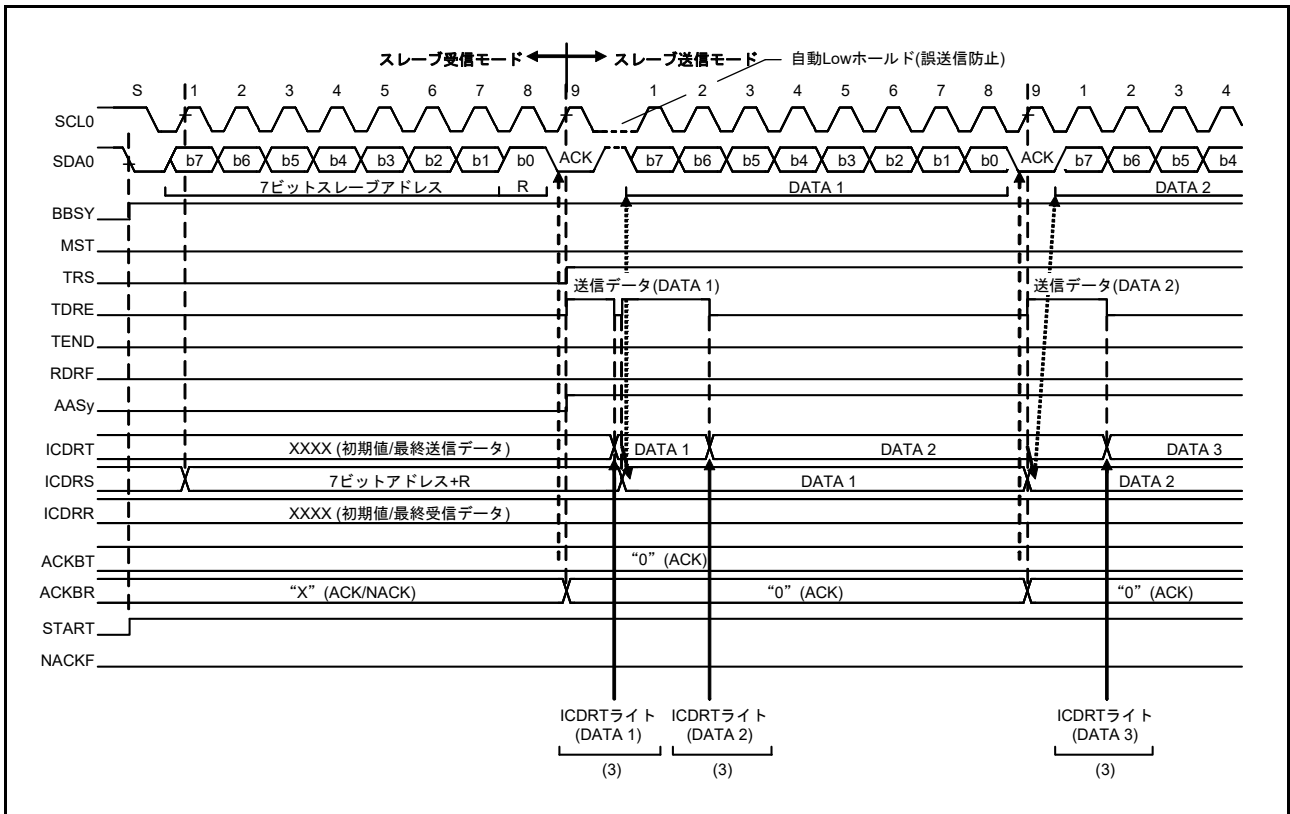
図 30.15 スレーブ送信の動作タイミング (1) (7ビットアドレスフォーマットの時)
