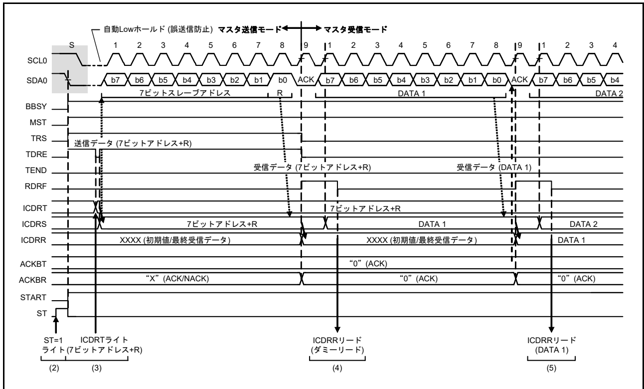
図 30.11 マスタ受信の動作タイミング (1) (7 ビットアドレスフォーマット、RDRFS ビット = 0 のとき)
