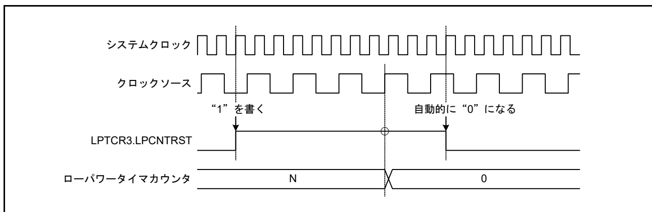
図 27.5 ローパワータイマカウンタのクリアタイミング
