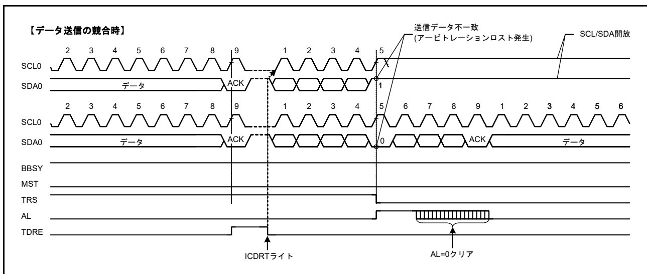
図 30.35 スレーブアービトレーションロスト検出動作例 (SALE ビット = 1 のとき)
