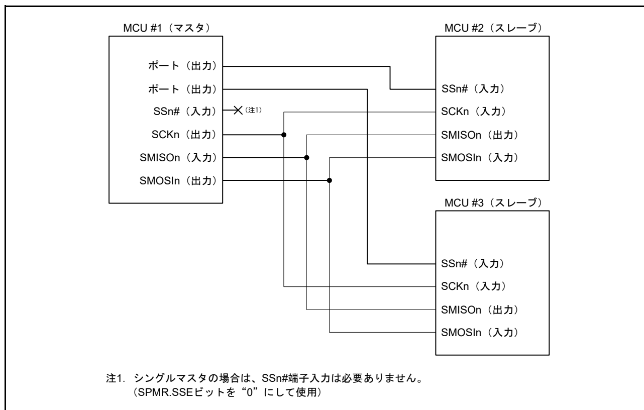
図 29.57 簡易 SPI モードの接続例 (シングルマスタ時 (SPMR.SSE ビット = 0))
