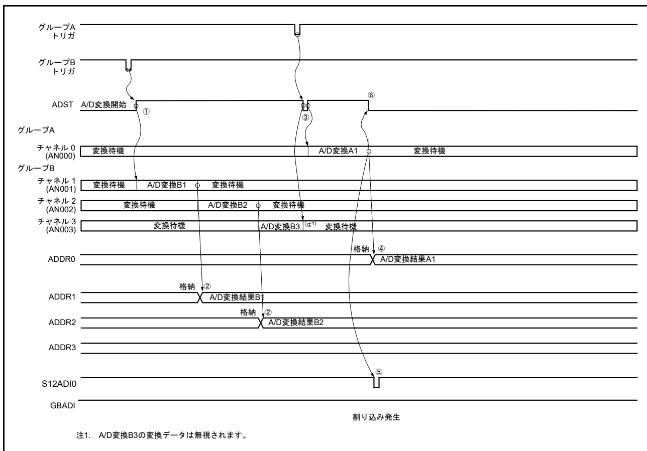
図 37.16 グループ A 優先制御の動作例 (4) (ADGSPCR.GBRSCN = 0, ADGSPCR.GBRP = 0 時の動作)
