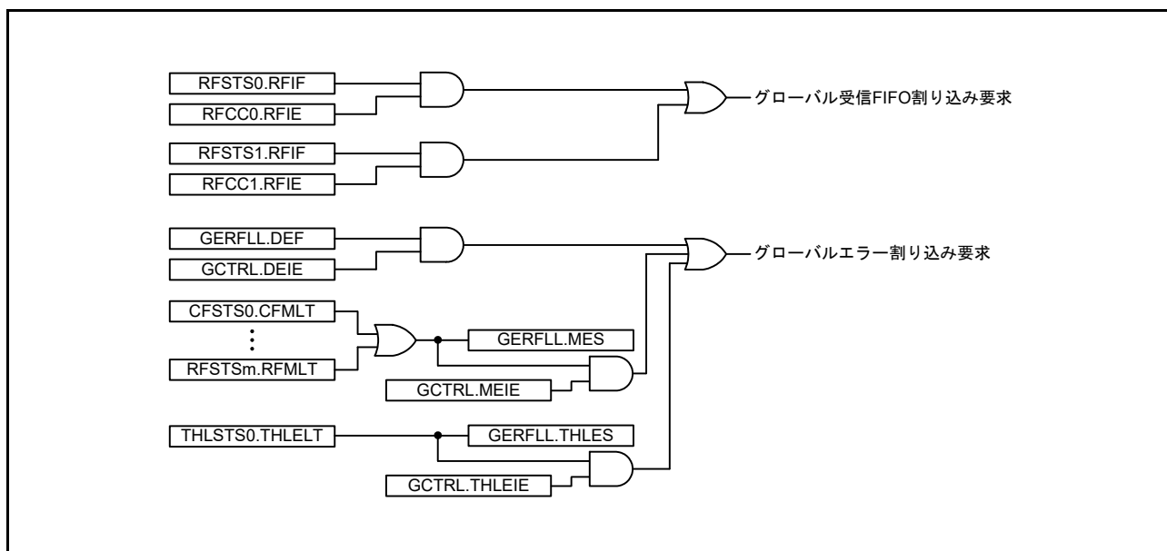
図 31.13 CAN グローバル割り込みブロック図
