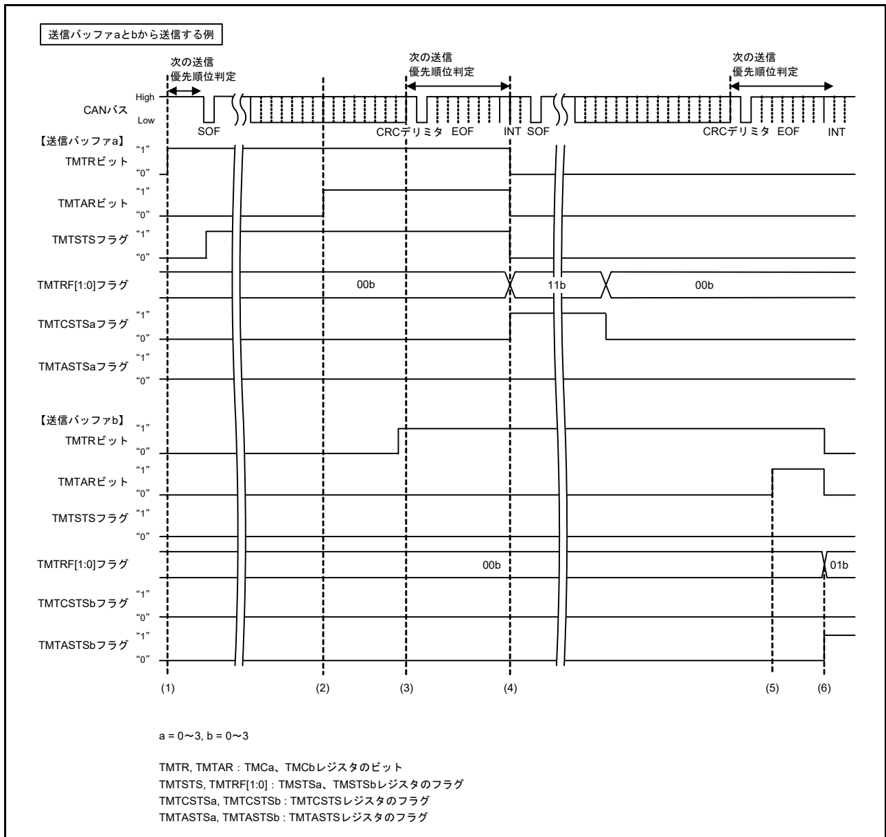
図 31.28 送信バッファの送信タイミング図 (送信アボート完了時)
