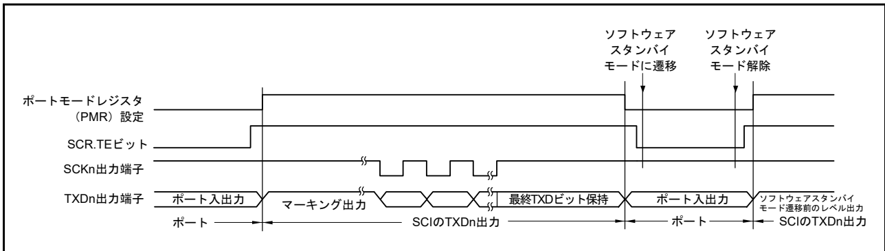
図 29.79 ソフトウェアスタンバイモード遷移時のポートの端子状態 (内部クロック、クロック同期送信)
