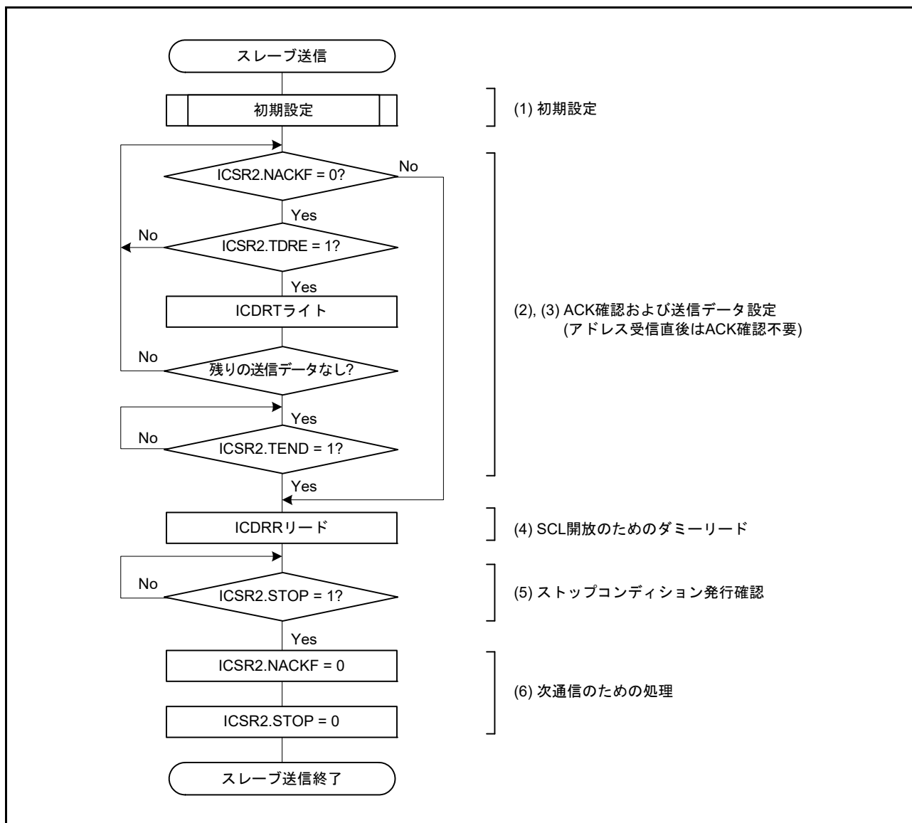
図 30.14 スレーブ送信のフローチャート例
