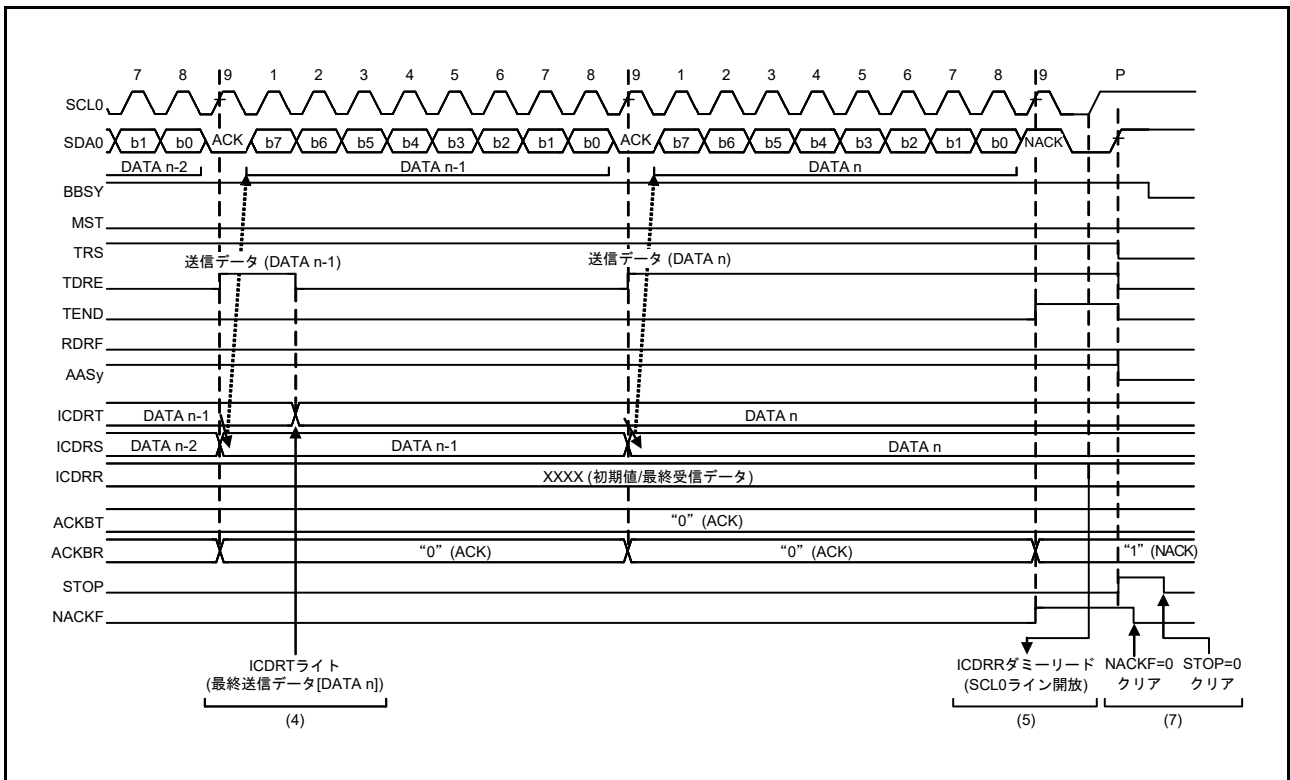
図 30.16 スレーブ送信の動作タイミング (2)
