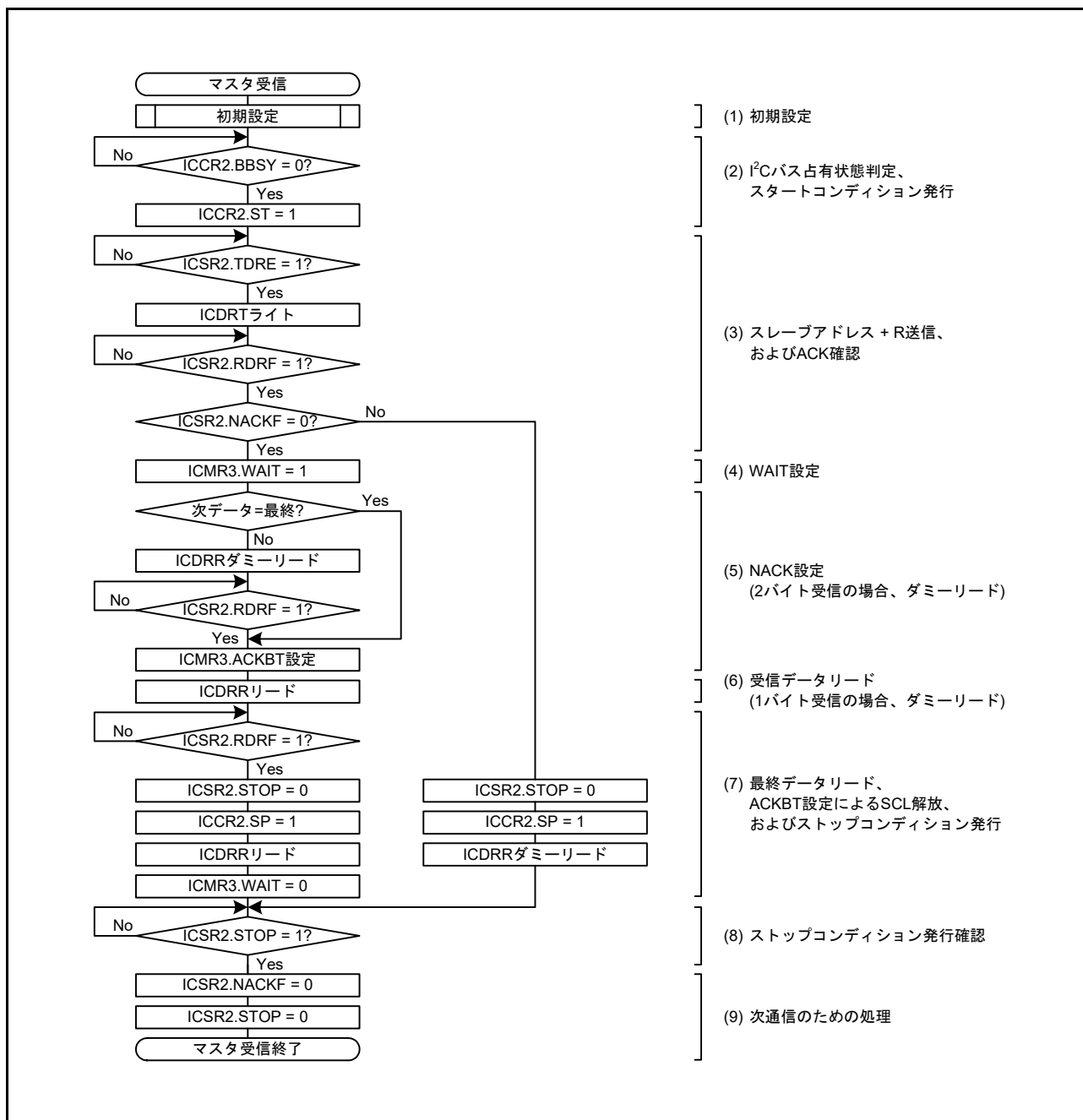
図 30.9 マスタ受信のフローチャート例 (7 ビットアドレスフォーマットの場合、2 バイト以下の場合)
