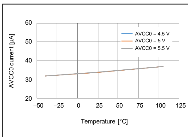
図 42.12 励起電流源動作電流の温度依存性
