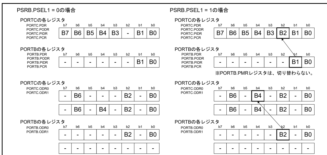
図 20.7 PSRBレジスタによる汎用入出力ポートの切り替え
