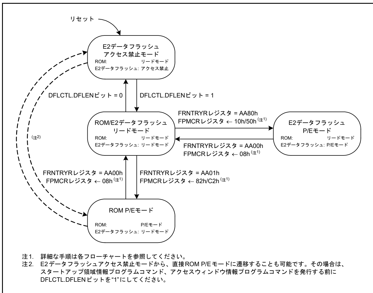
図 41.6 フラッシュメモリのモード遷移図
