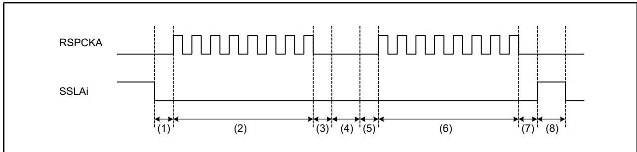
図 32.36 SSLKP ビットを利用したバースト転送動作の例 (CPHA = 1, CPOL = 0)
