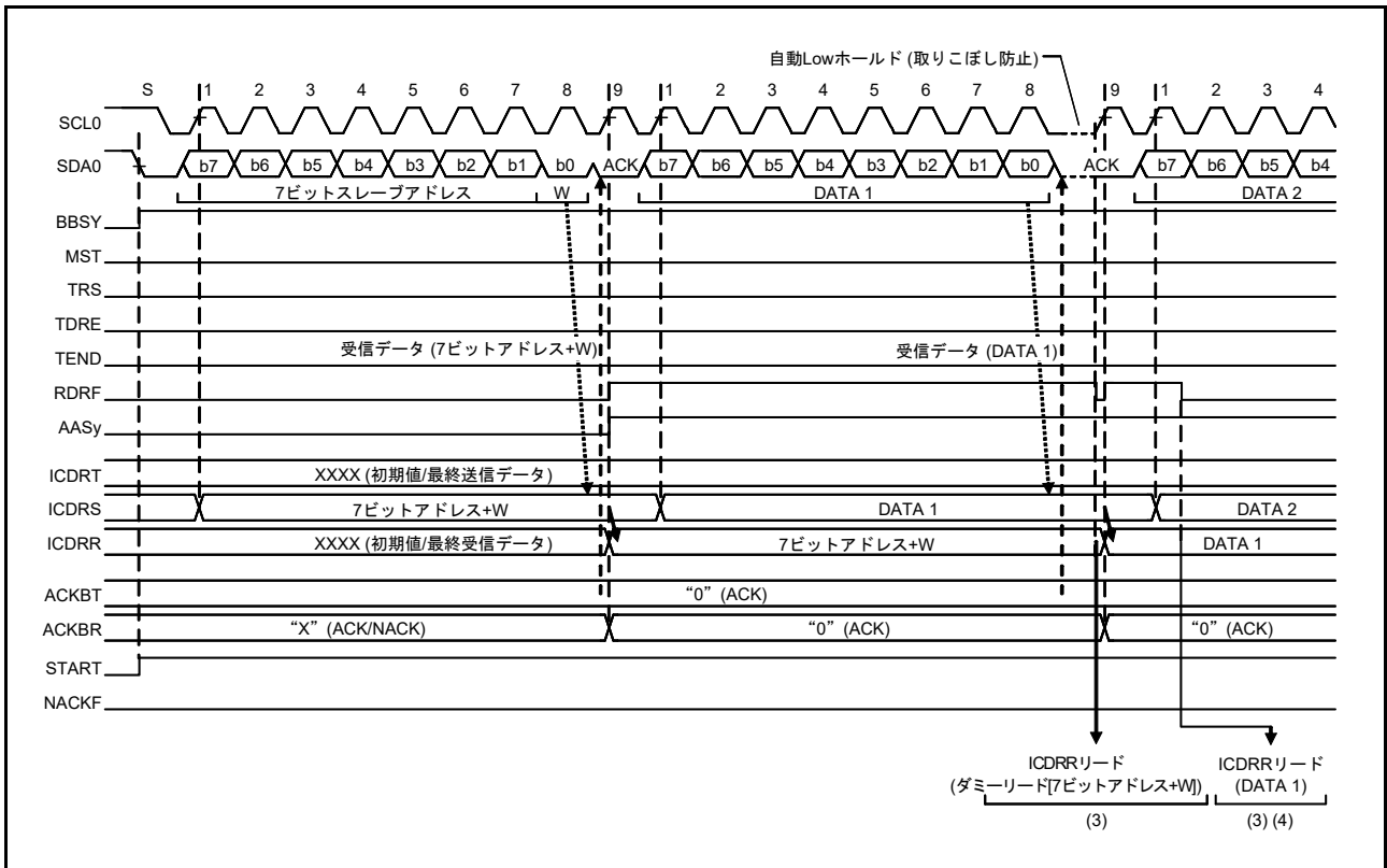
図 30.18 スレーブ受信の動作タイミング (1) (7ビットアドレスフォーマット、RDRFS ビット = 0 のとき)
