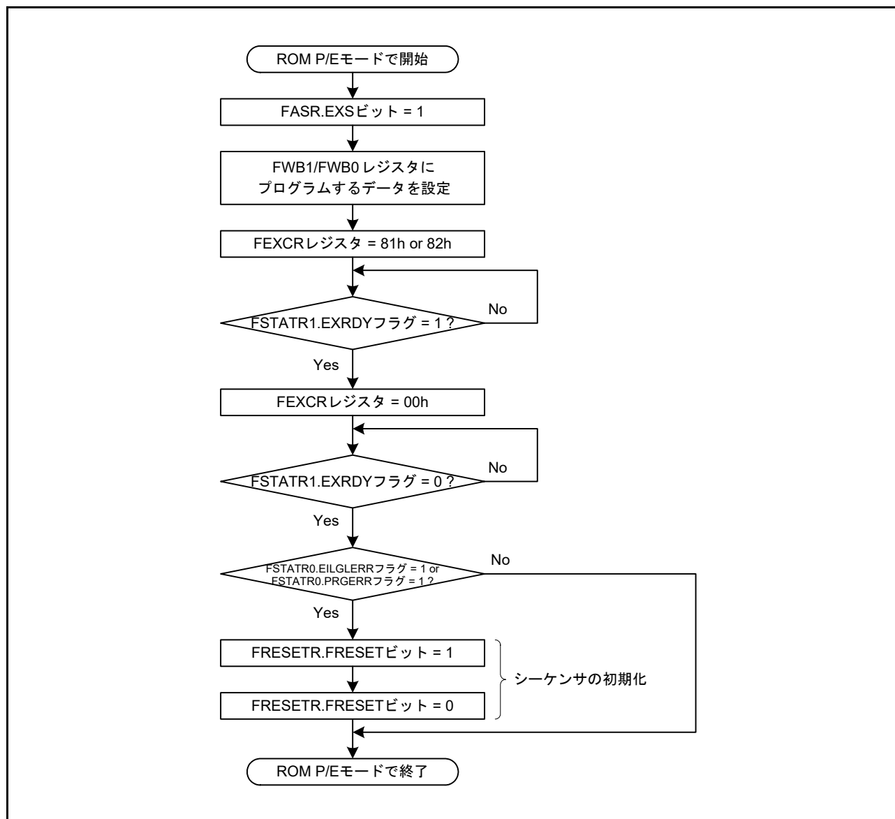
図 41.20 スタートアップ領域情報プログラムコマンド/アクセスウィンドウ情報プログラムコマンドの発行フロー
