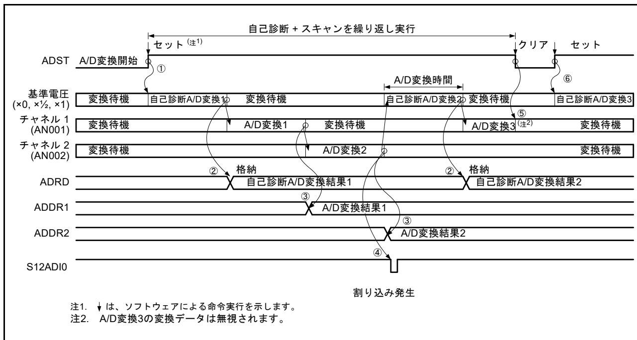
図 37.9 連続スキャンモードの動作例 (基本動作 : AN001、AN002 選択 + 自己診断)
