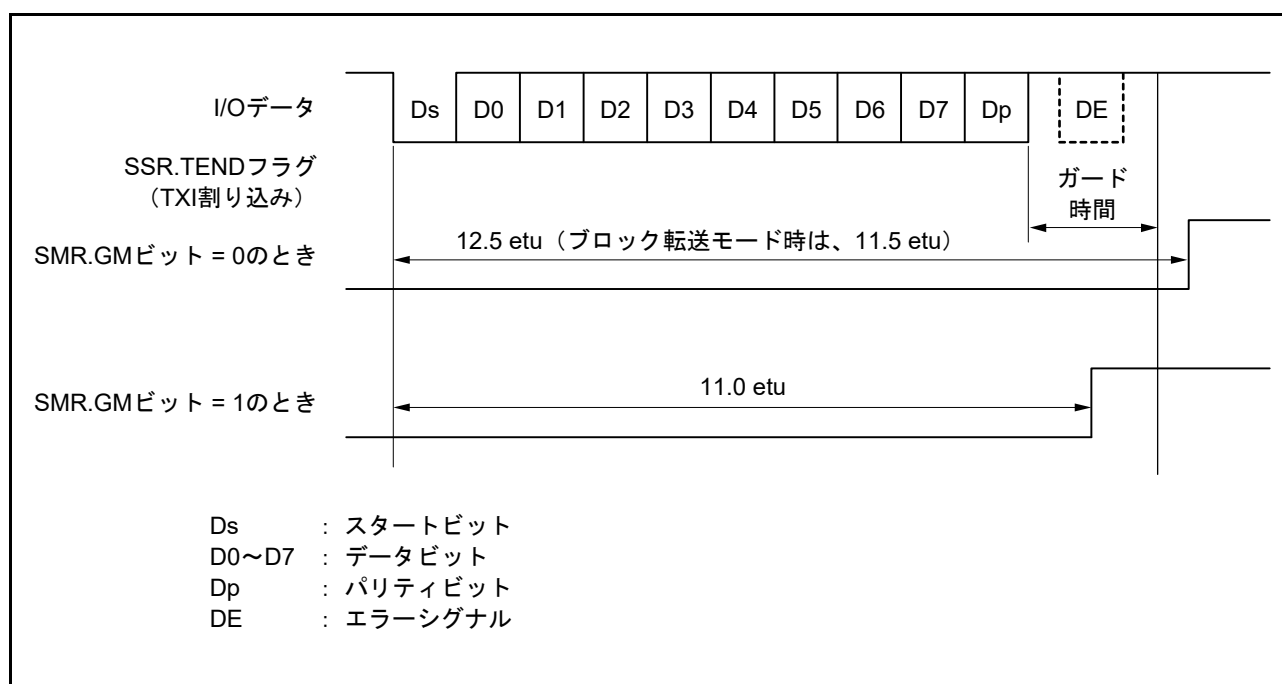
図 29.42 送信時の SSR.TEND フラグの発生タイミング
