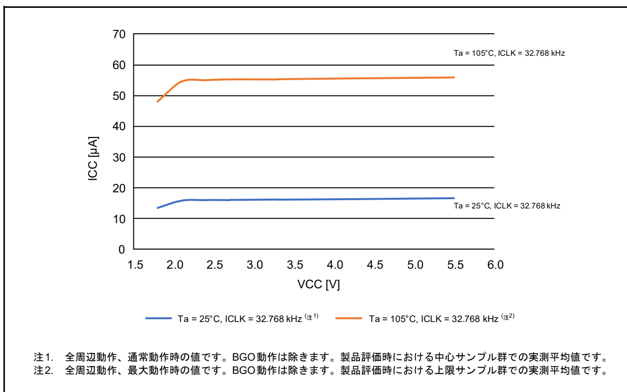
図 42.3 低速動作モードの電圧依存性 (参考データ)
