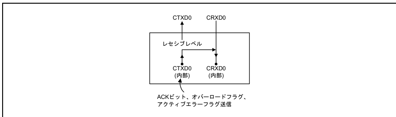
図 31.10 リッスンオンリモード選択時の接続
