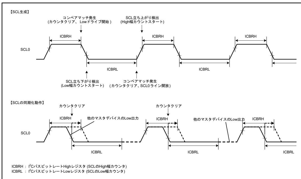
図 30.20 RIIC の SCL 生成および SCL 同期化動作
