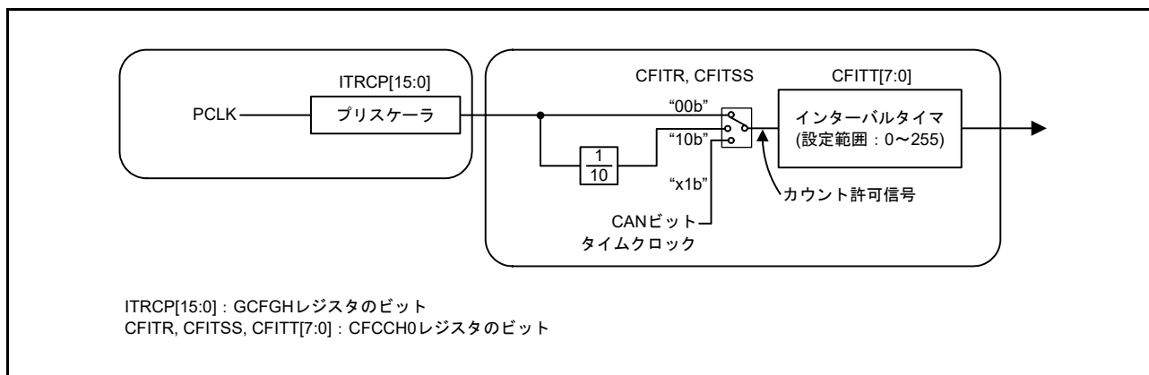
図 31.8 インターバルタイマのブロック図
