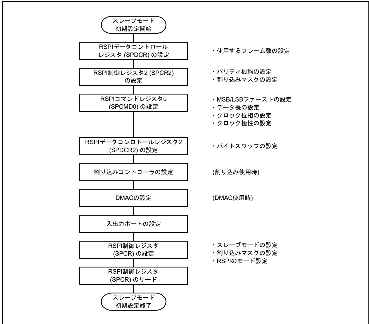
図 32.49 スレーブモード時の初期化フロー例 (クロック同期式動作)
