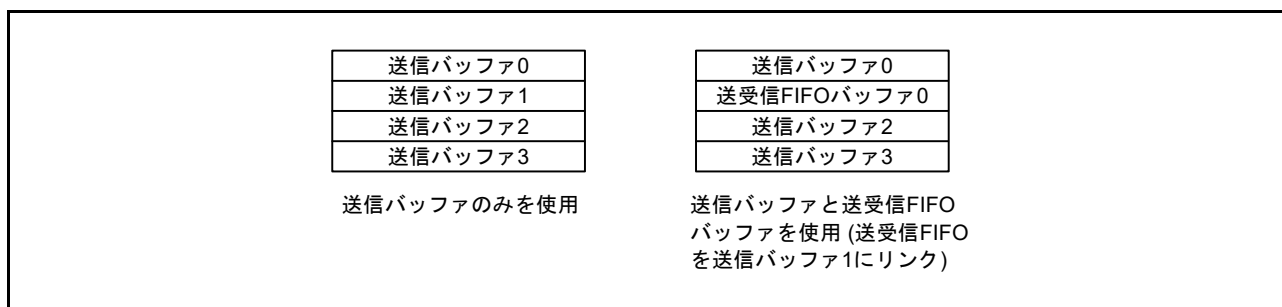
図 31.7 送受信 FIFO バッファのリンク
