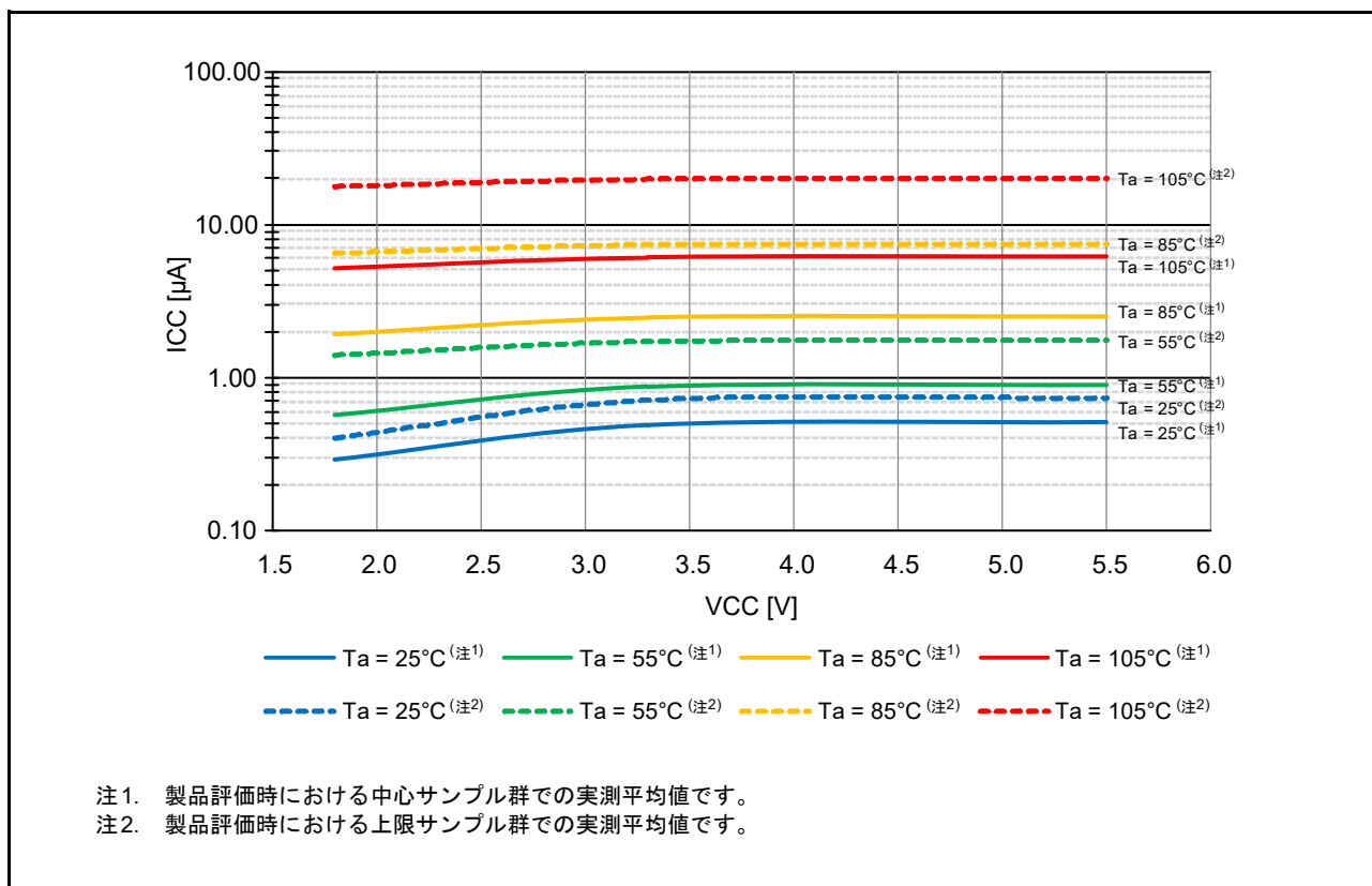
図 42.4 ソフトウェアスタンバイモード時の電圧依存性 (参考データ)
