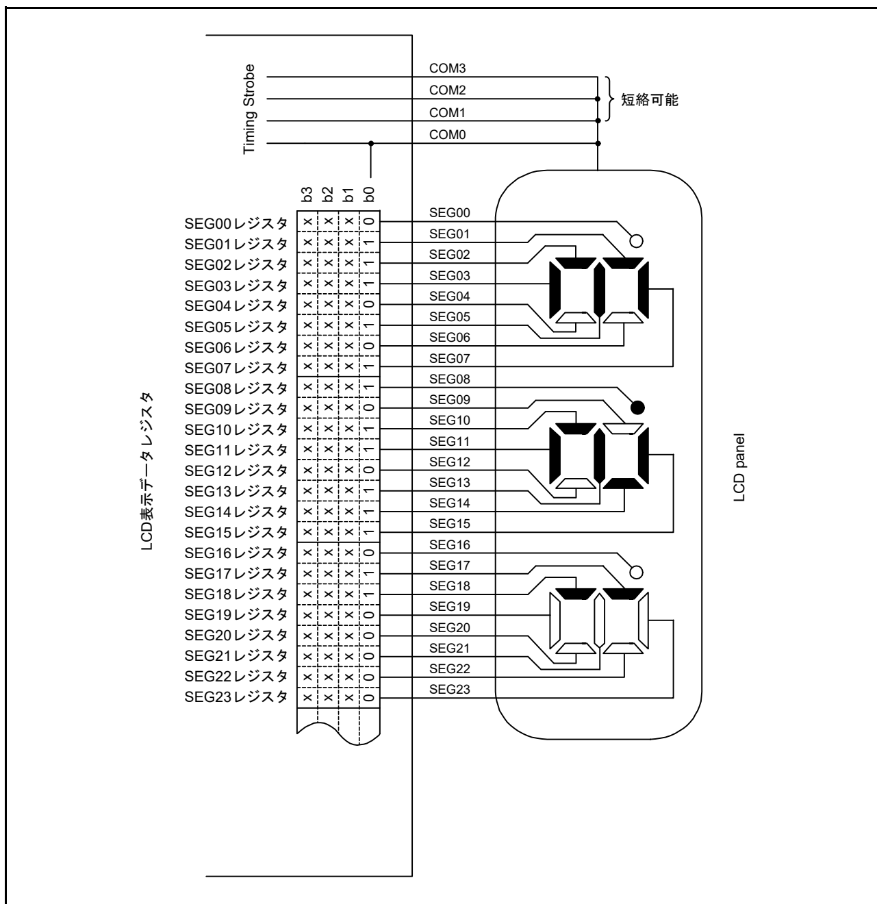
図 34.19 スタティック LCD パネルの結線例
