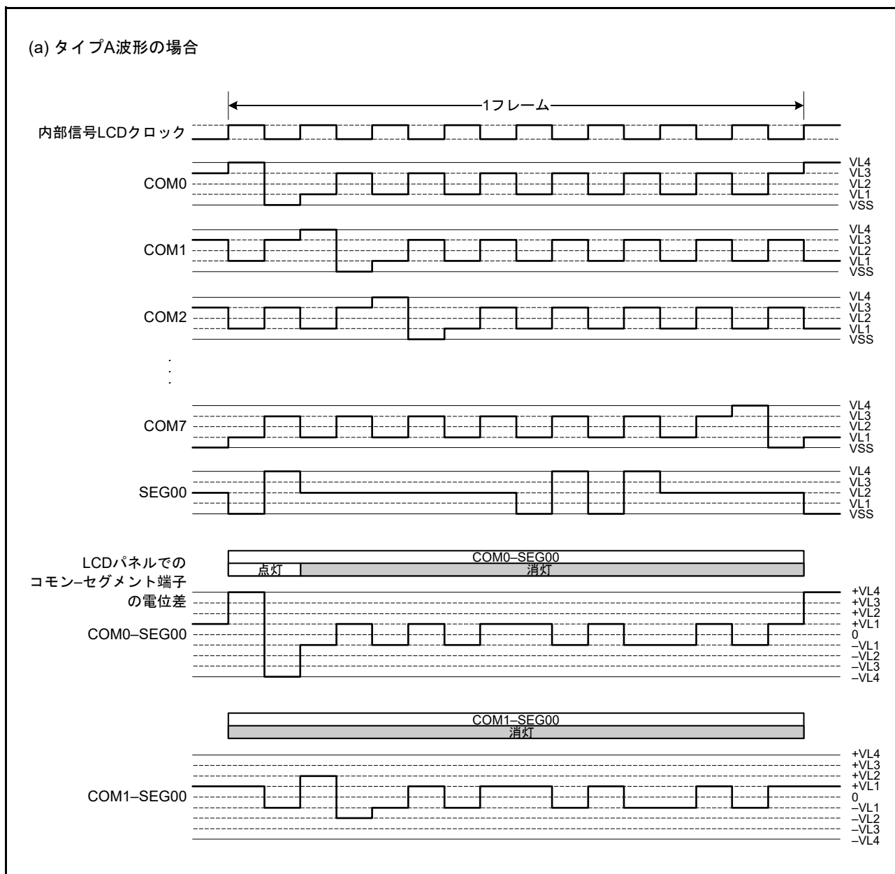
図 34.34 SEG00 端子と各コモン端子間の 1/8 デューティ LCD 駆動波形例 (1/4 バイアス) (1)
