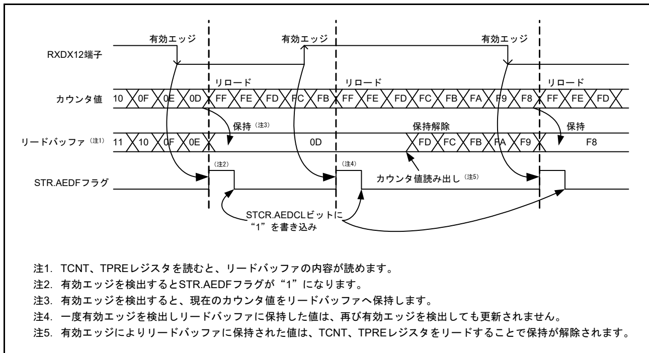
図 29.71 ビットレート測定機能動作例
