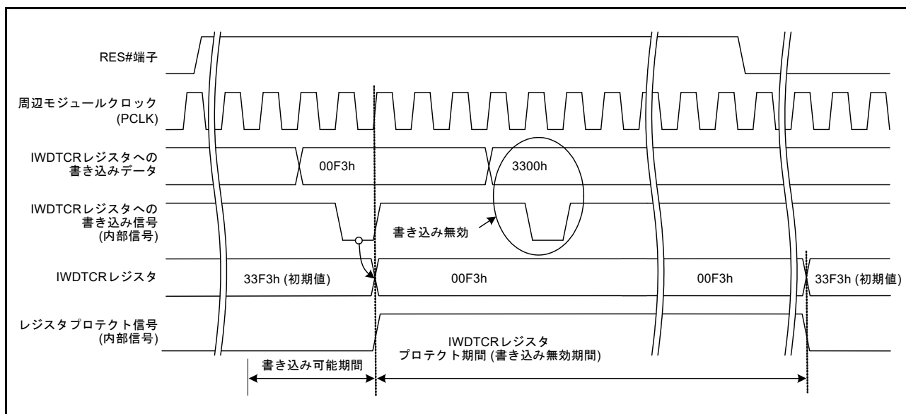
図 28.5 IWDTCR レジスタ書き込み制御波形
