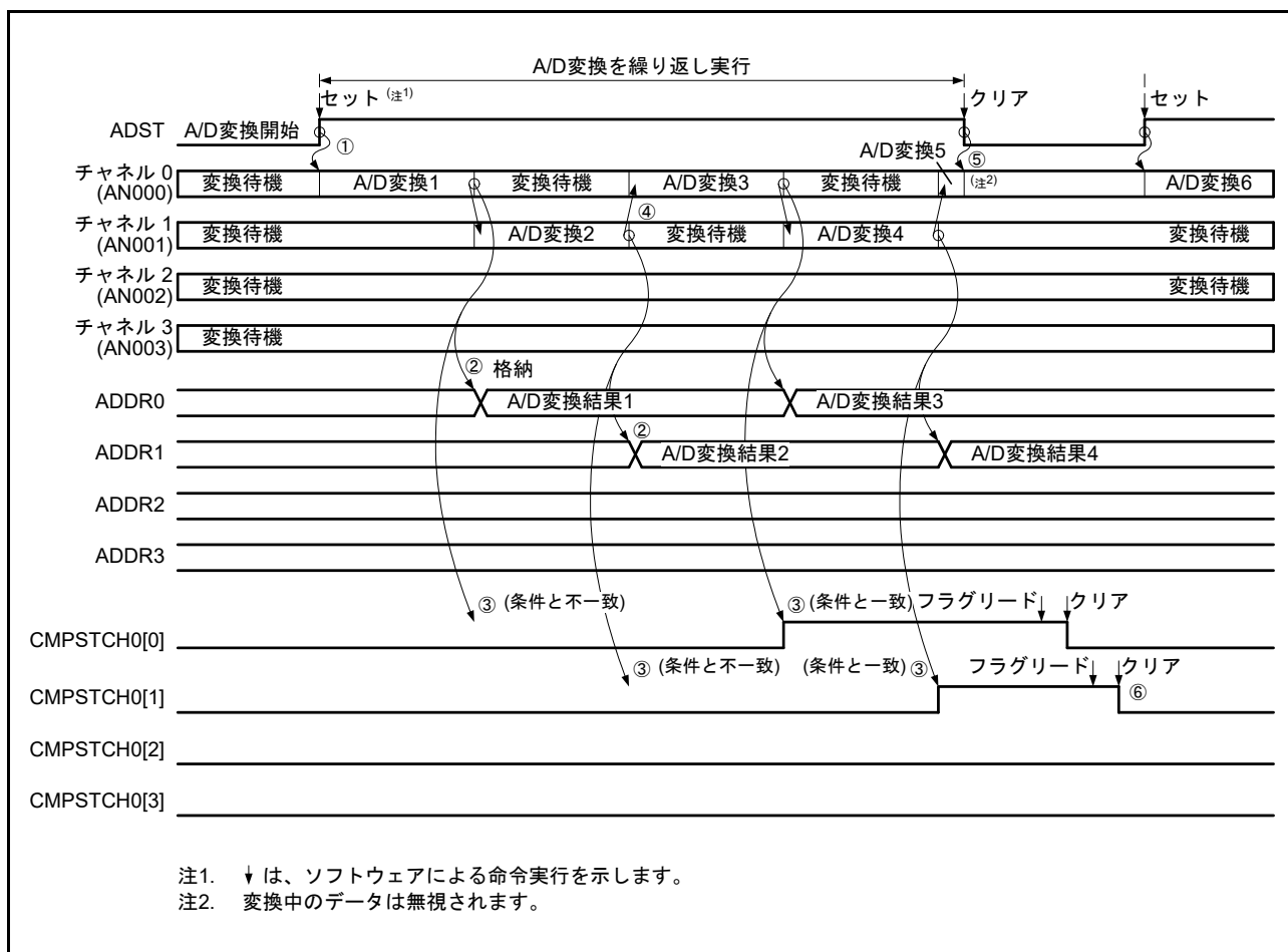
図 37.18 コンペア機能の動作例 (AN000、AN001、AN002、AN003 コンペア対象)
