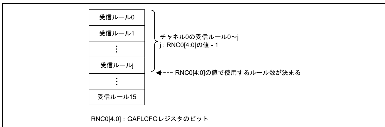
図 31.4 受信ルール登録
