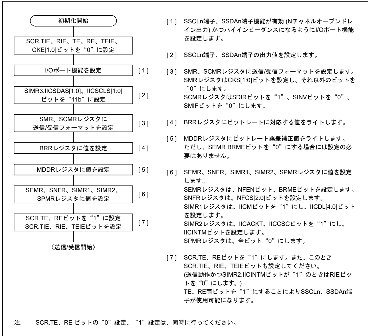
図 29.51 SCI の初期化フローチャート例 (簡易 I 2 C モード)
