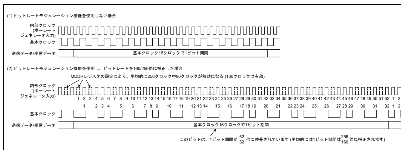
図 29.59 ビットレートモジュレーション機能使用時の基本クロックの例
