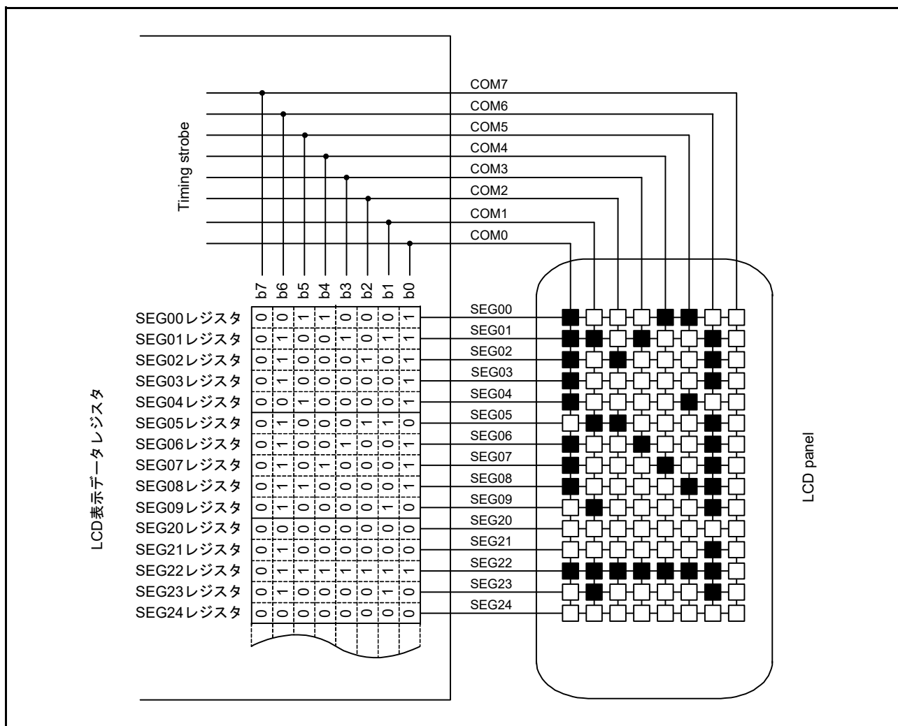
図 34.33 1/8 デューティ LCD パネルの結線例
