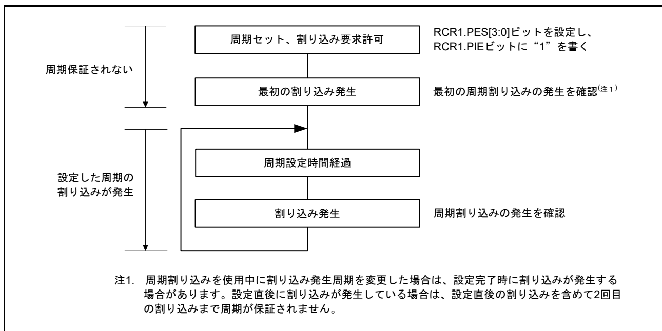
図 26.11 周期割り込み機能の使用方法
