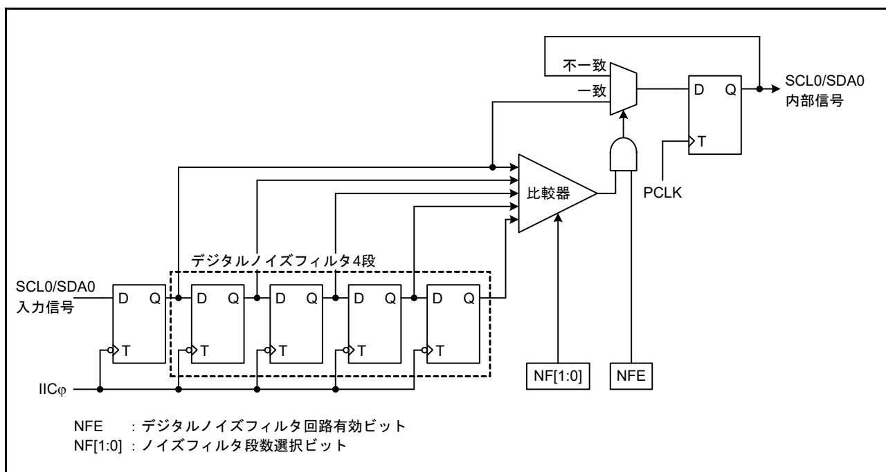
図 30.22 デジタルノイズフィルタ回路のブロック図
