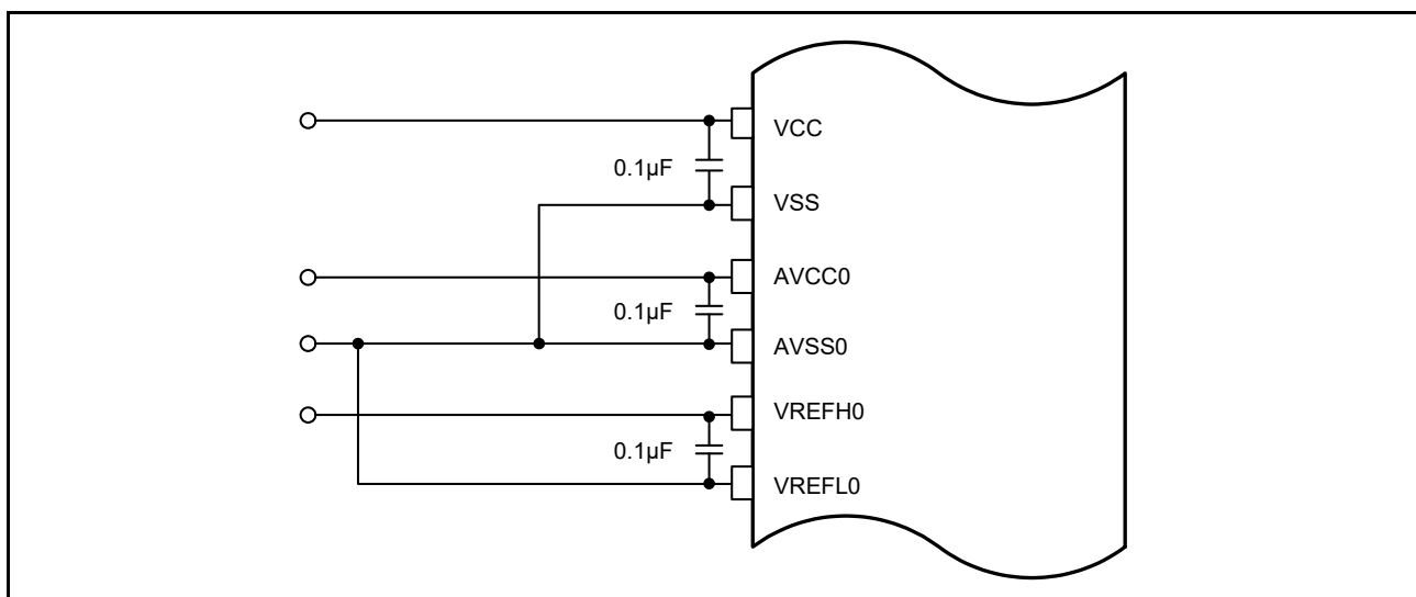
図 37.30 各電源端子の接続例
