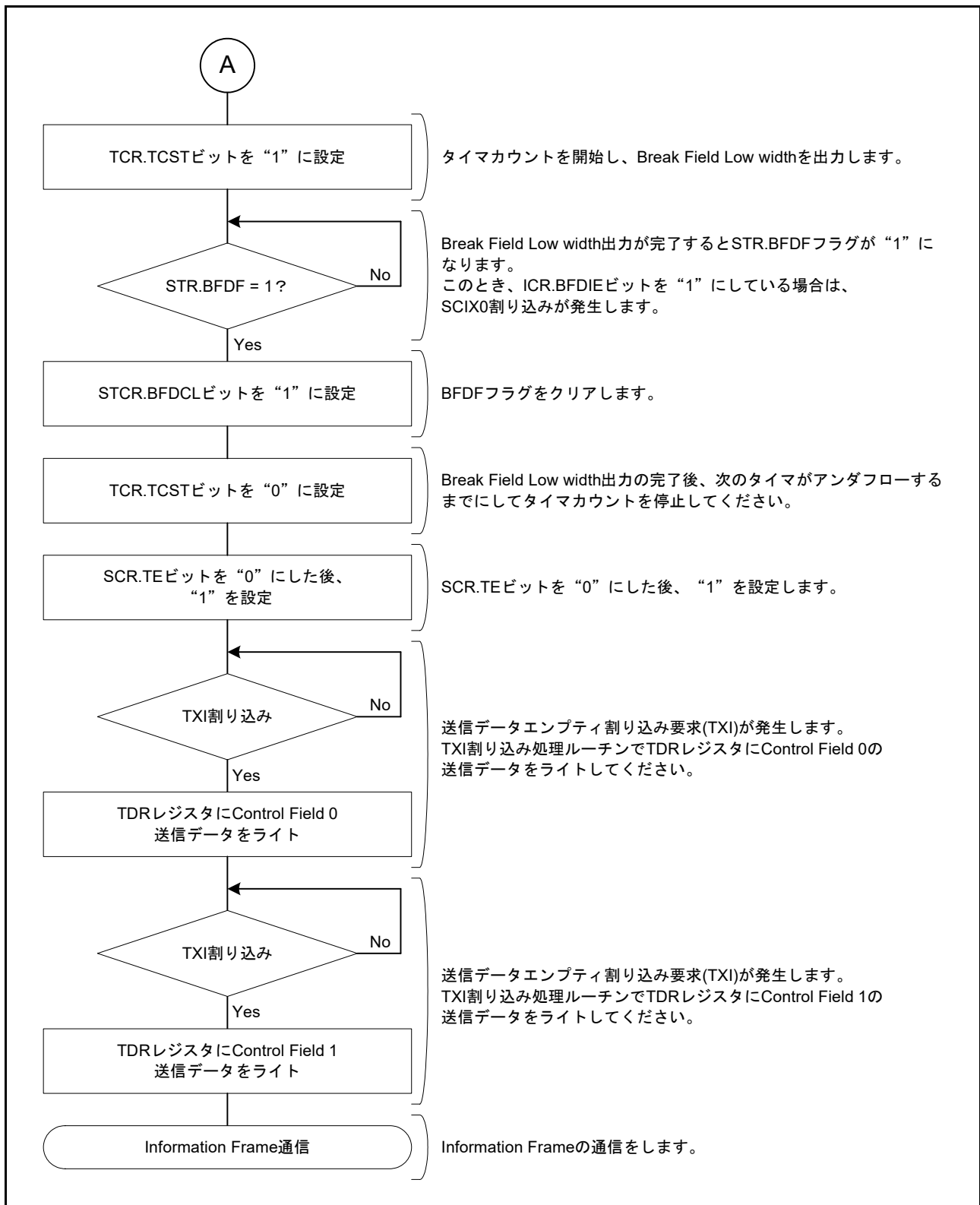
図 29.63 Start Frame 送信フローチャート例 (2)
