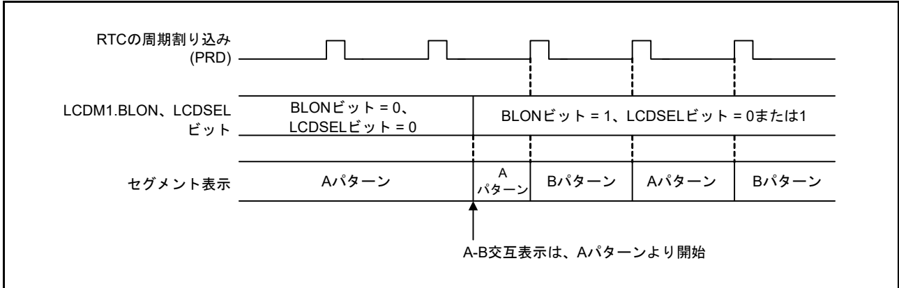
図 34.3 Aパターン領域表示から A-B 交互表示への切り替え動作
