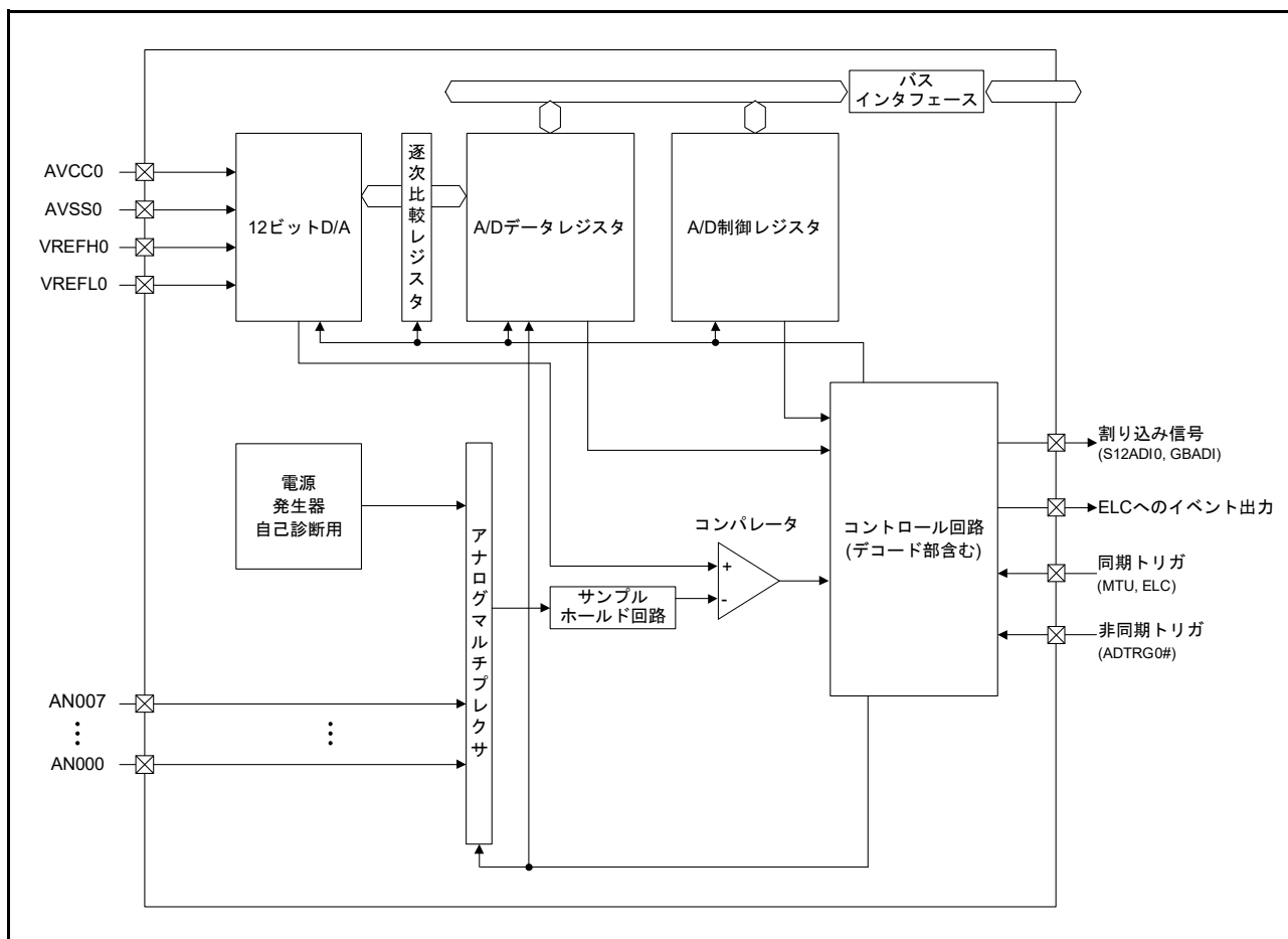
図 37.1 12ビットA/Dコンバータのブロック図
