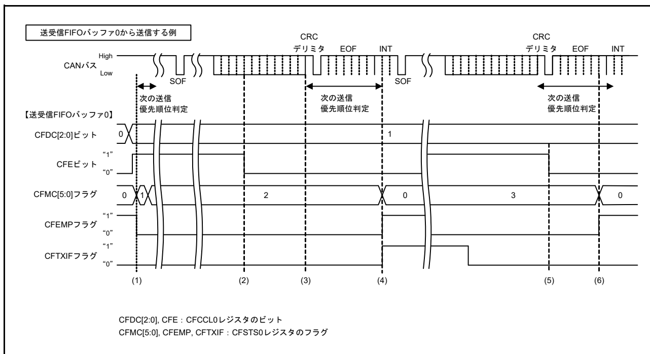
図 31.31 送受信 FIFO バッファの送信タイミング図 (送信アポート完了時)
