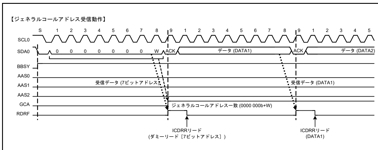
図 30.26 ジェネラルコールアドレス受信時に GCA フラグが “1” になるタイミング
