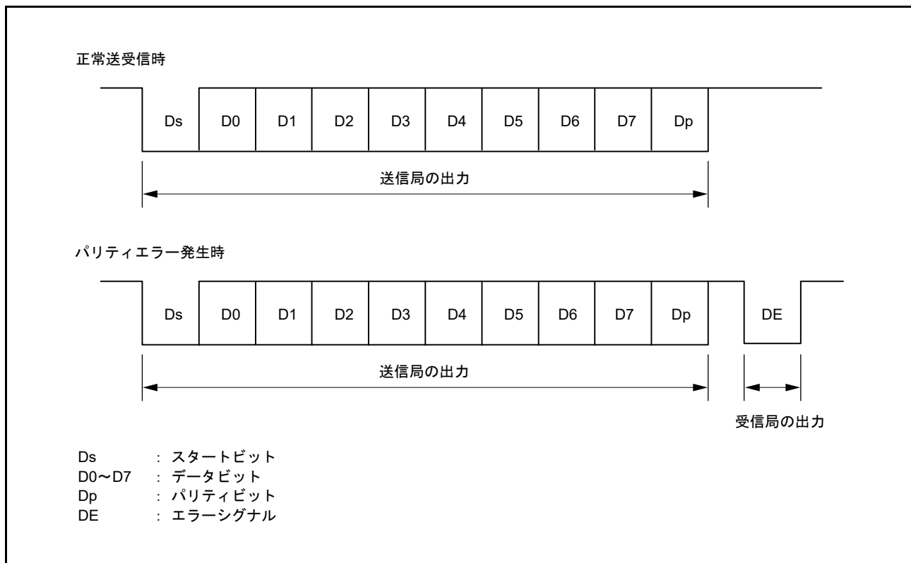
図 29.34 スマートカードインタフェースモードのデータフォーマット
