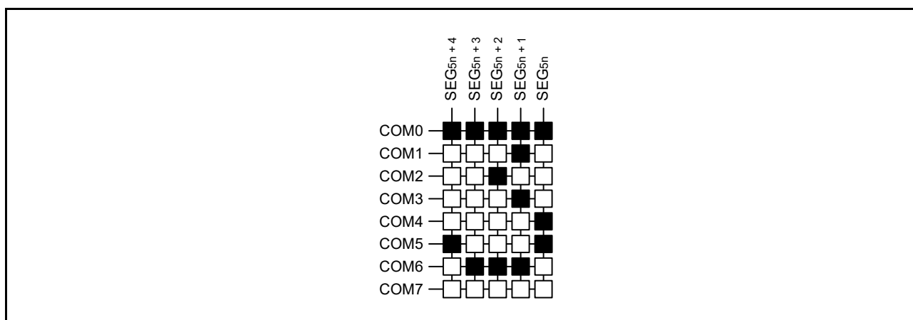
図 34.32 1/8 デューティ LCD の表示パターンと電極結線 (n = 0, 1, 4)
