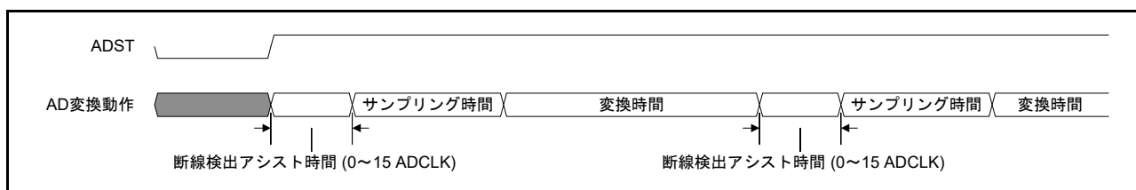
図 37.23 断線検出アシスト機能を使用した場合の A/D 変換動作図
