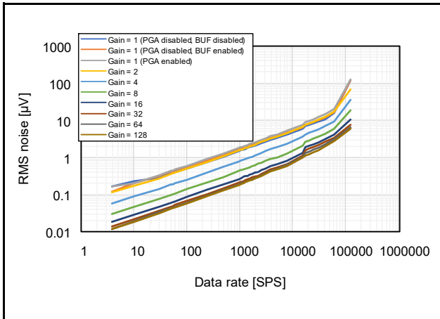
図 42.67 RMS ノイズのデータレート依存性 (AVCC0 = 5.0V、 T_a = 25^\circ\text{C} 、 f_{\text{MOD}} = 4\text{MHz} 、Sinc 4 フィルタまたは Sinc 4 +Sinc 4 フィルタ、 V_{\text{ID}} = 0\text{V} 、 V_{\text{REF}} = 2.5\text{V} 、リファレンスバッファ無効)
