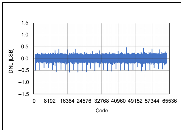
図 42.98 微分非直線性誤差のコード依存性 (AVCC0 = 5V, VREFH = 5V, T_a = 25^\circ\text{C} )
