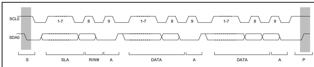
図 30.3 I 2 C バスタイミング (SLA = 7 ビットの場合)
