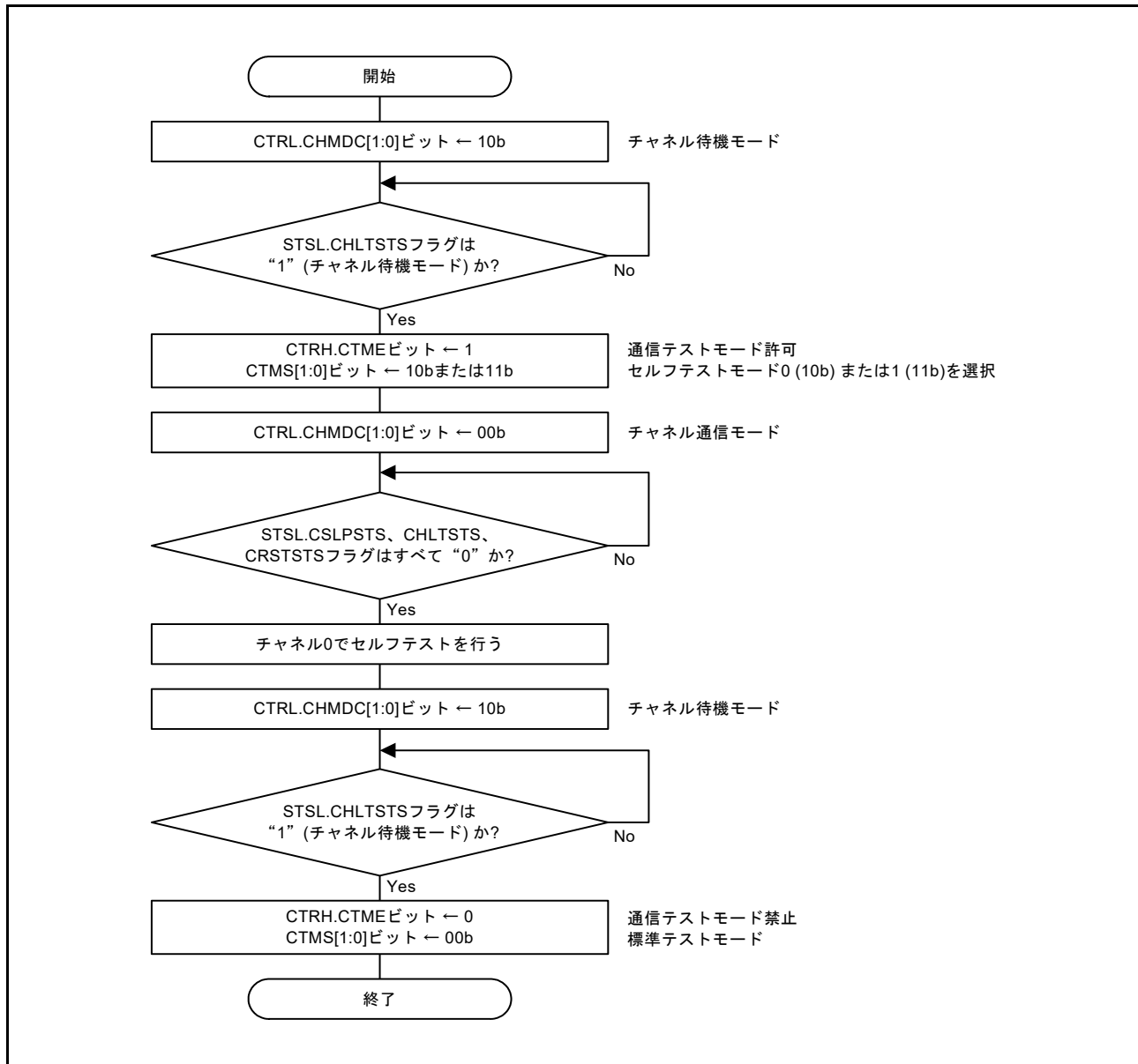
図 31.33 セルフテストモードの設定手順
