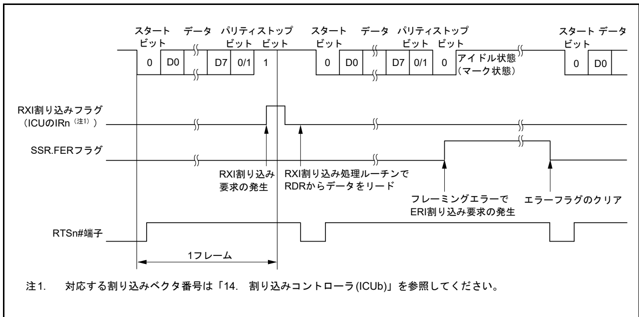
図 29.15 調歩同期式モードのシリアル受信時の動作例 (2) (RTS 機能使用時) (8ビットデータ / パリティあり / 1ストップビットの例)
