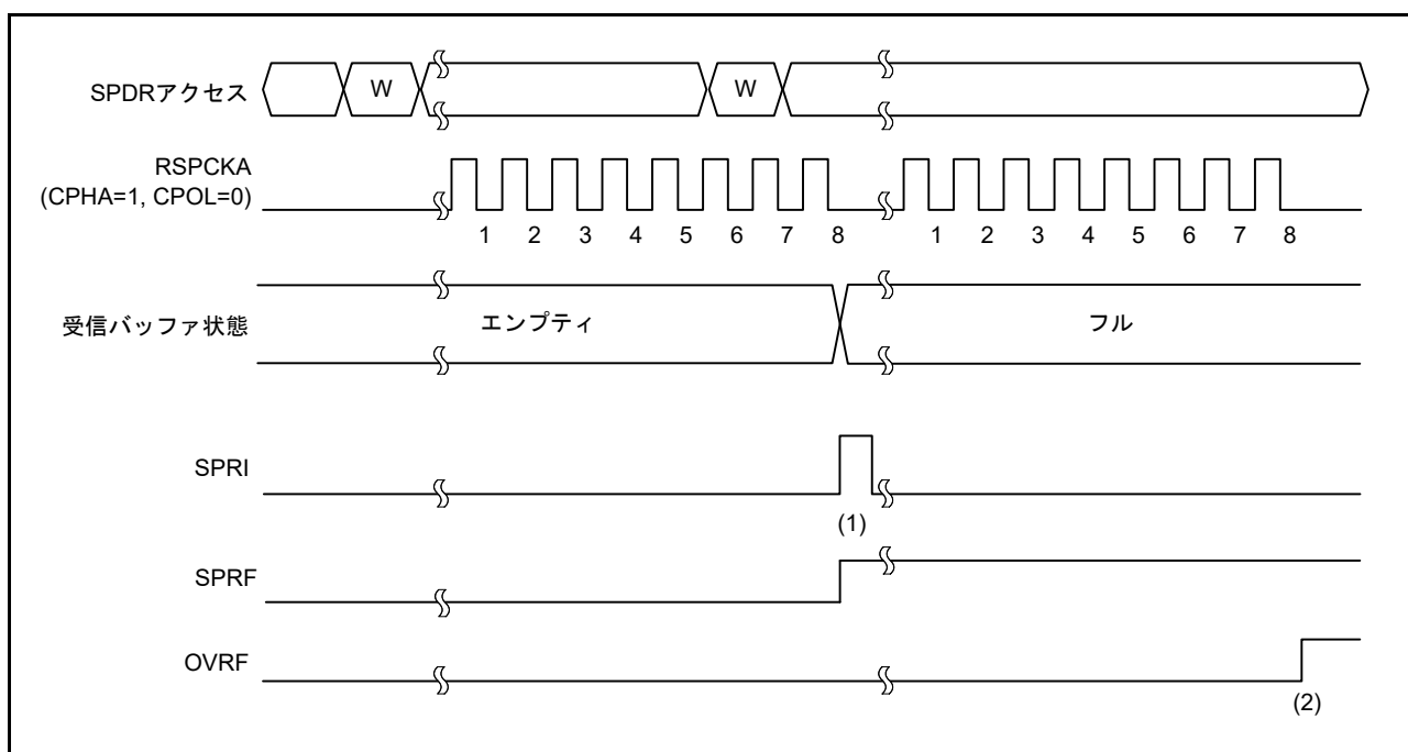
図 32.26 SPCR.TXMD = 0 の動作例
