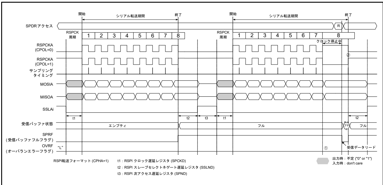
図 32.30 マスタモードの受信バッファフル状態でシリアル転送が継続するときのクロック停止波形 (CPHA = 1)
