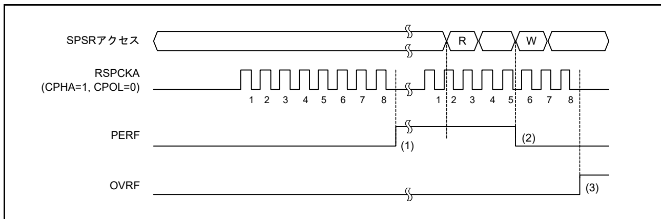
図 32.32 PERF フラグの動作例
