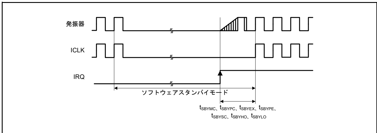
図 42.27 ソフトウェアスタンバイモード復帰タイミング
