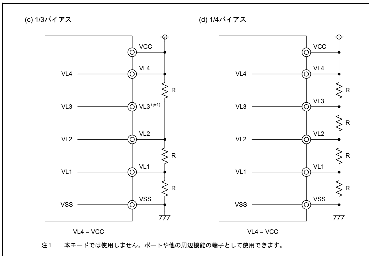
図 34.10 LCD バイアス電圧の供給例 (外部抵抗分割方式) (2)
