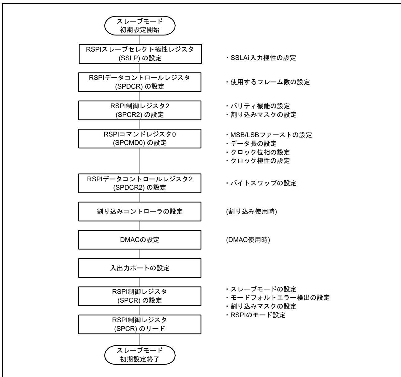
図 32.41 スレーブモード時の初期化フロー例 (SPI 動作)
