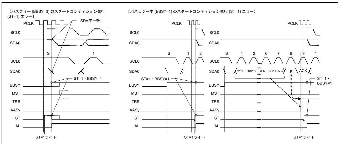
図 30.33 スタートコンディション発行時のアービトレーションロスト (MALE ビット = 1 のとき)
