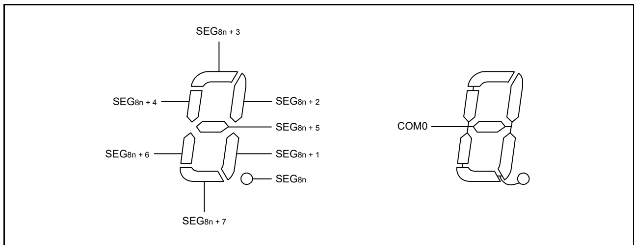
図 34.18 スタティック LCD の表示パターンと電極結線 (n = 0 ~ 2)
