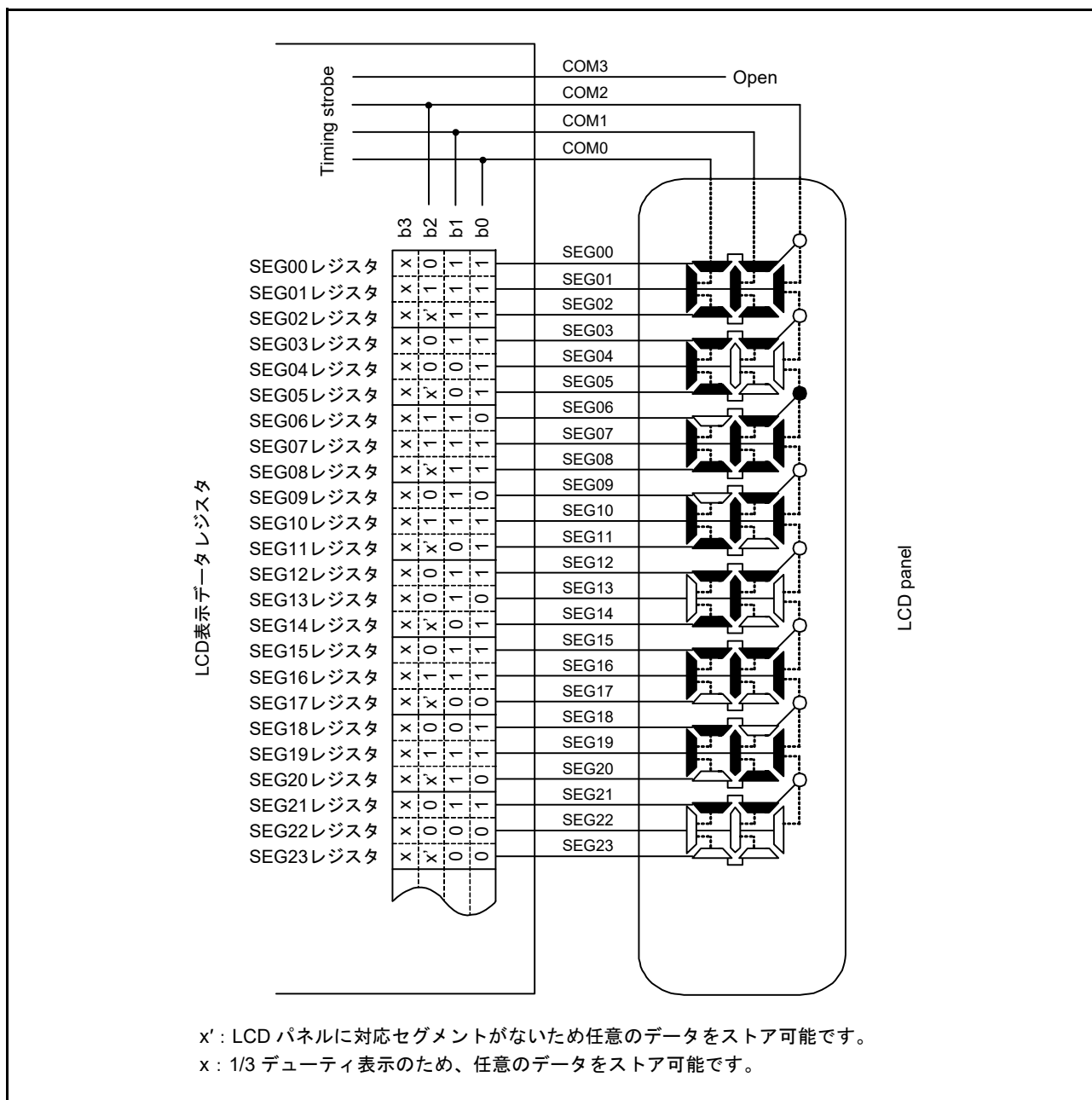
図 34.25 1/3 デューティ LCD パネルの結線例
