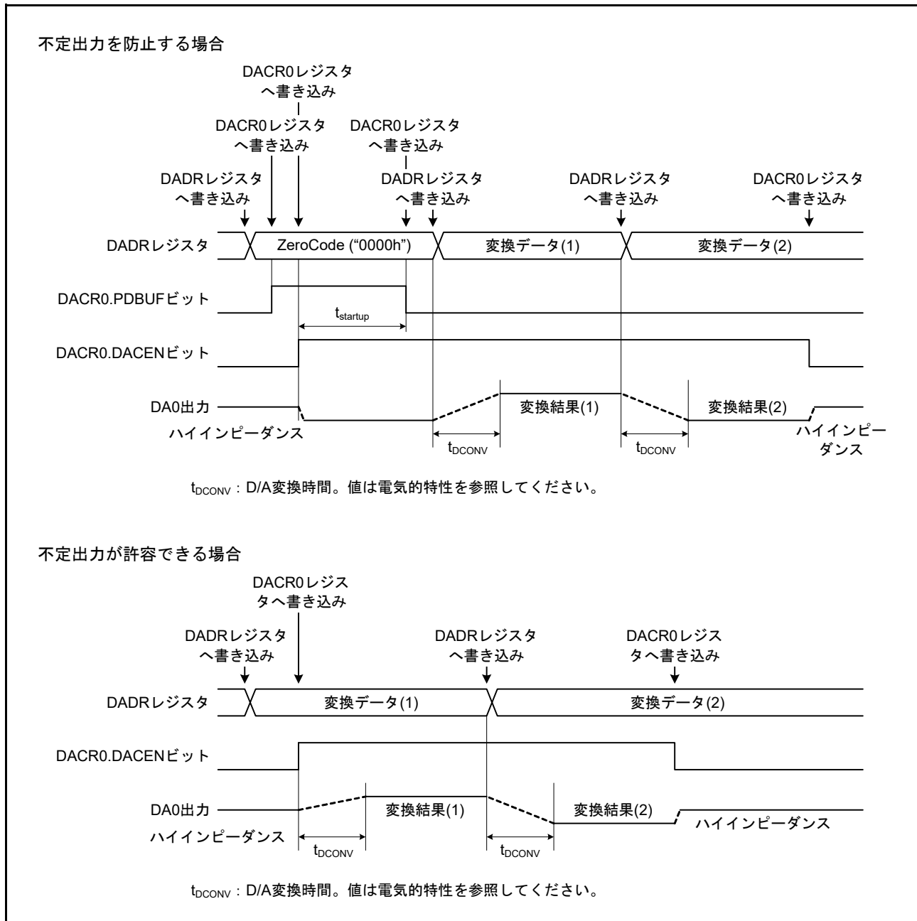
図 38.2 16ビットD/Aコンバータの動作例
