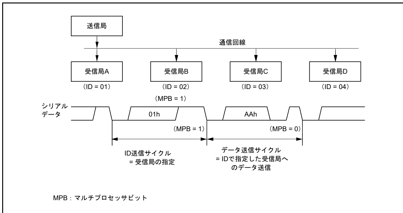
図 29.18 マルチプロセッサフォーマットを使用した通信例 (受信局 A へのデータ“AAh”の送金の例)
