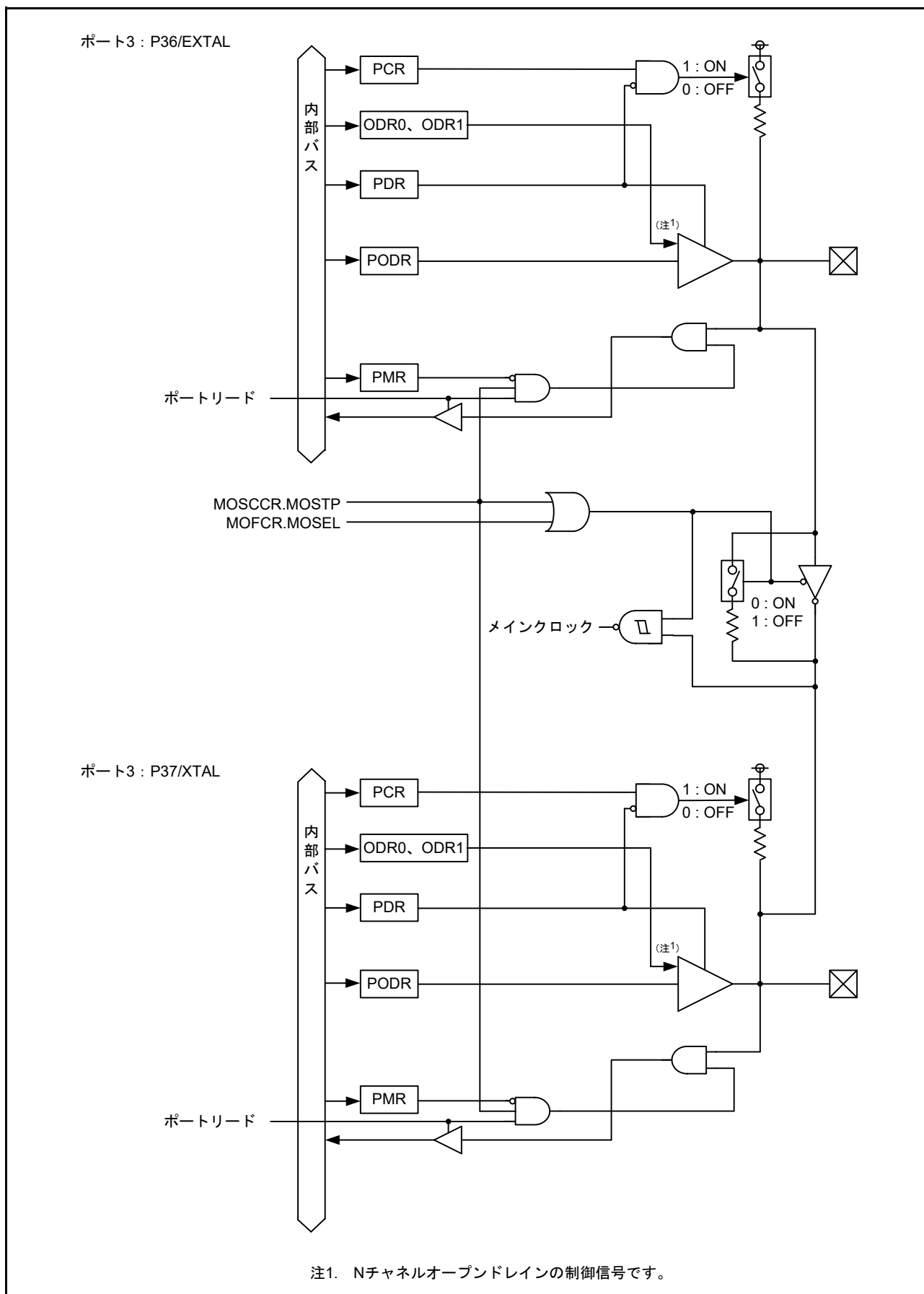
図 20.3 入出力ポートの構成 (3)
