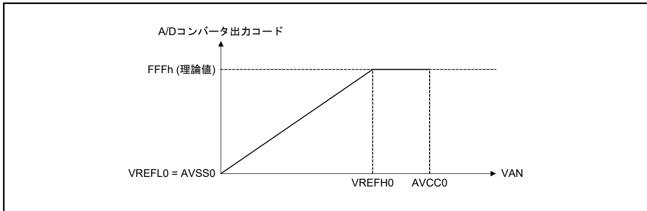
図 37.29 アナログ入力端子に印加する電圧と出力コードの関係
