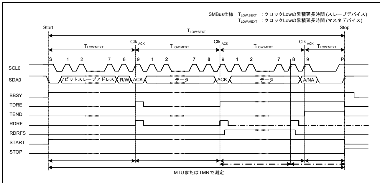
図 30.40 SMBus タイムアウト測定
