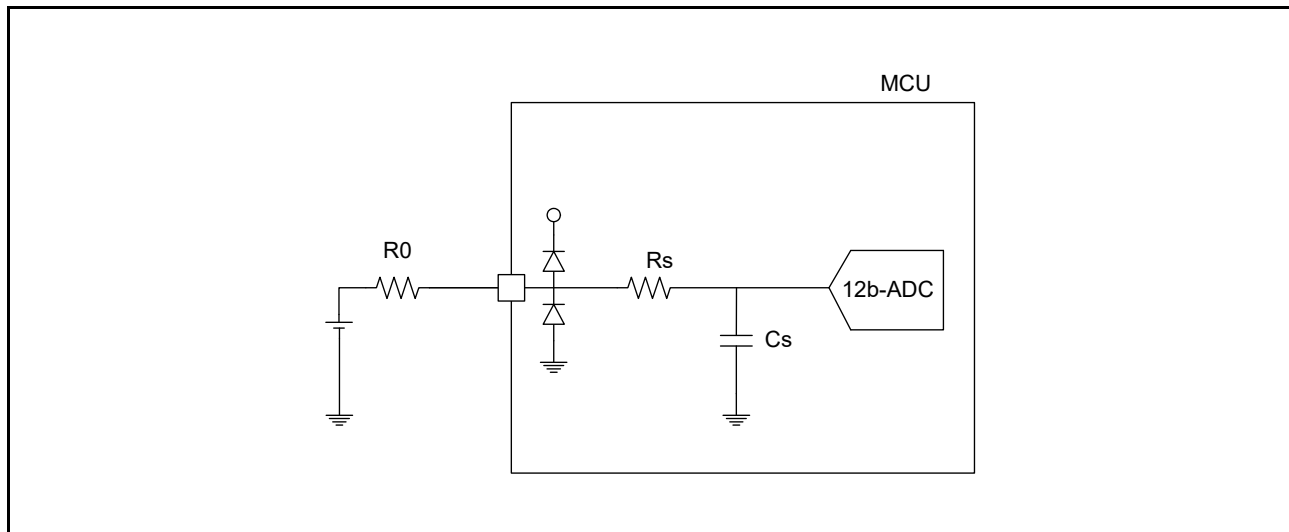
図 42.95 等価回路
