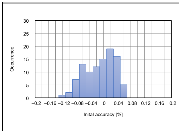
図 42.83 基準電圧源初期精度 (AVCC0 = 5.0V)
