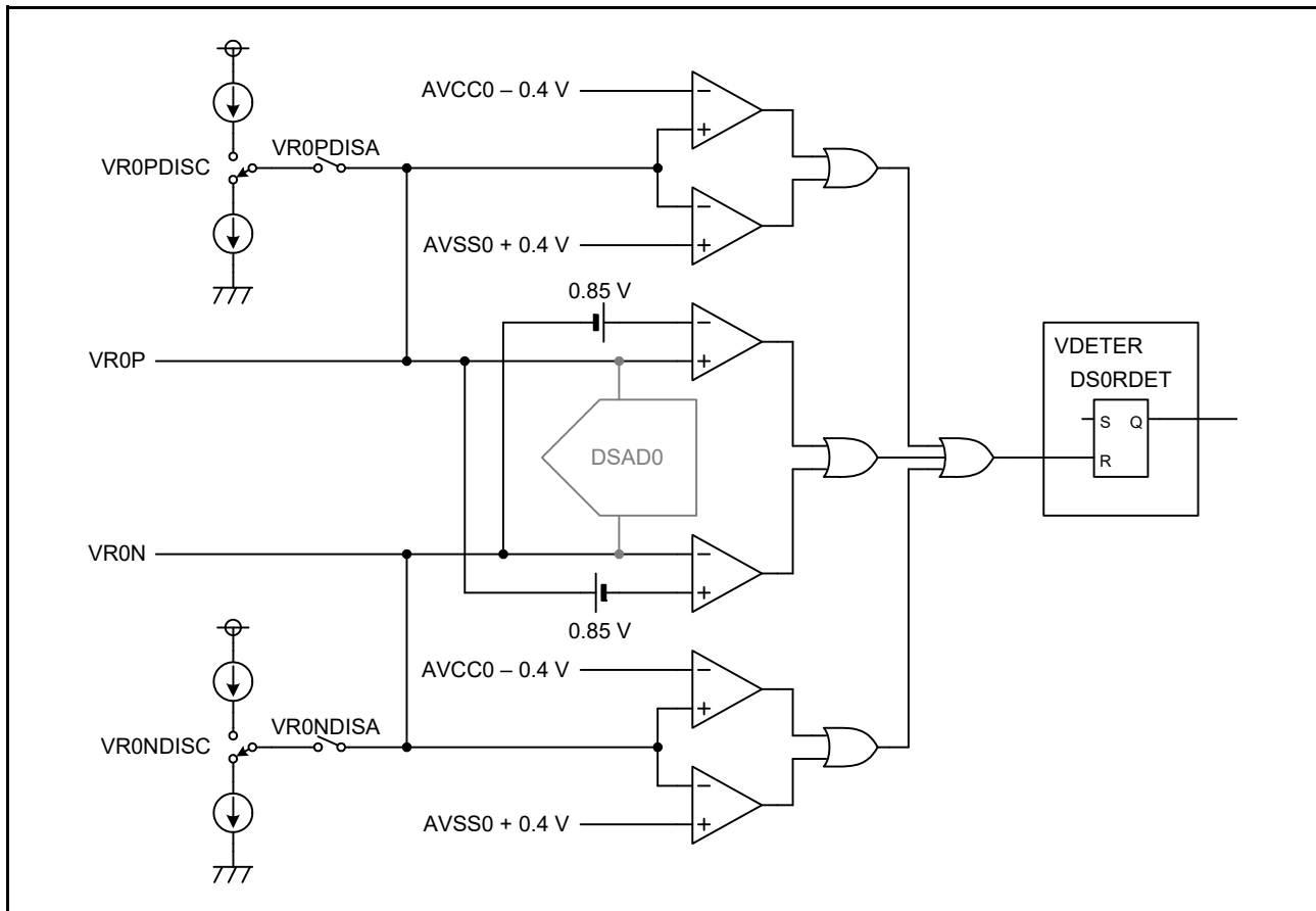
図 35.12 DSRDET のブロック図
