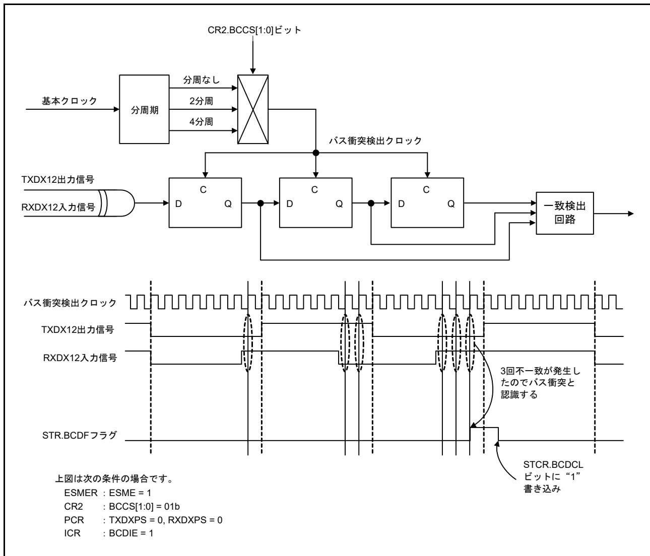
図 29.69 バス衝突検出機能の動作例
