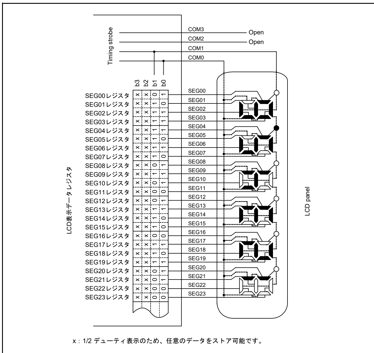
図 34.22 1/2 デューティ LCD パネルの結線例
