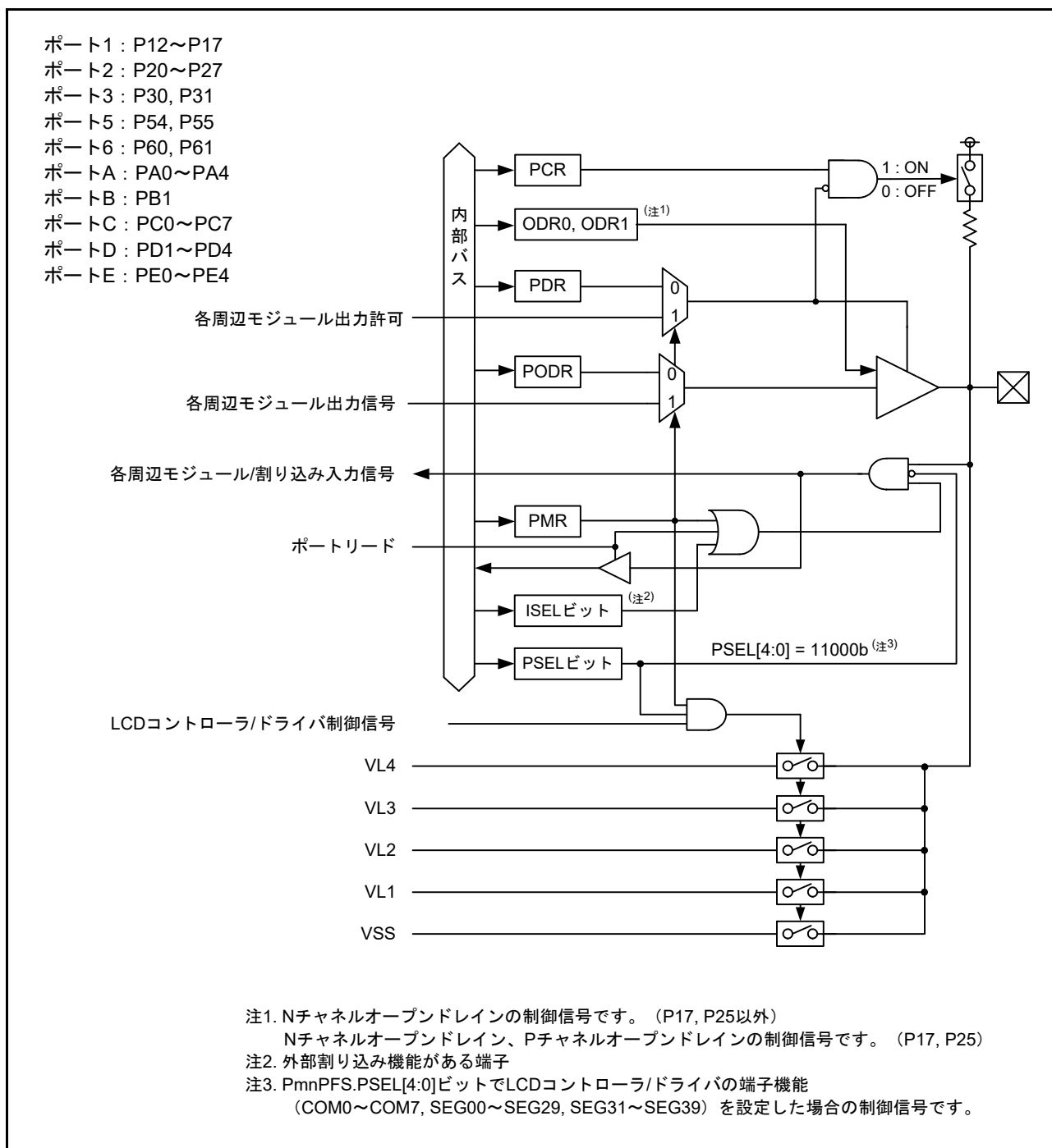
図 20.1 入出力ポートの構成 (1)
