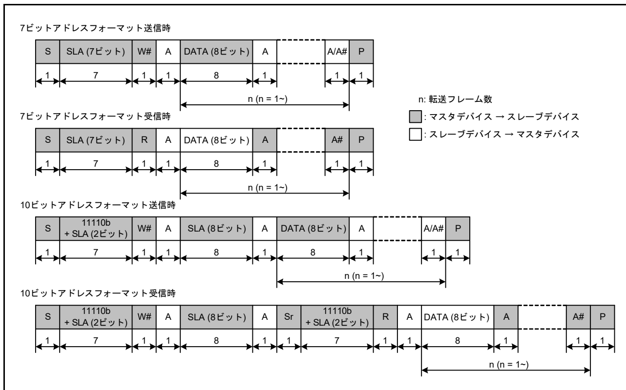
図 29.46 I 2 C バスフォーマット
