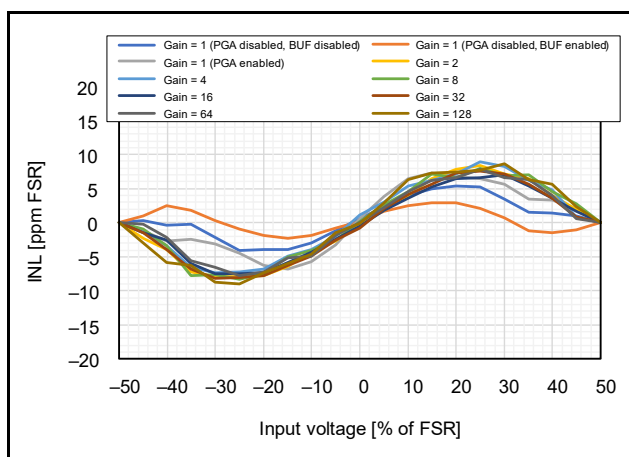
図 42.69 積分非直線性誤差の入力電圧依存性 (AVCC0 = 5.0V、 T_a = 25^\circ\text{C} 、 f_{\text{MOD}} = 4\text{MHz} 、総合 OSR = 4096、 V_{\text{REF}} = 2.5\text{V} )
