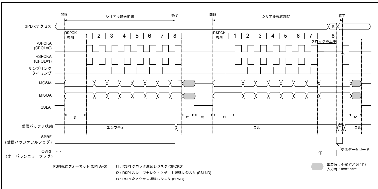
図 32.31 マスタモードの受信バッファフル状態でシリアル転送が継続するときのクロック停止波形 (CPHA = 0)
