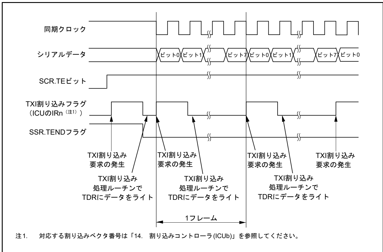
図 29.25 クロック同期式モードのシリアル送信の動作例 (1) (送信開始・CTS 機能使用しない)
