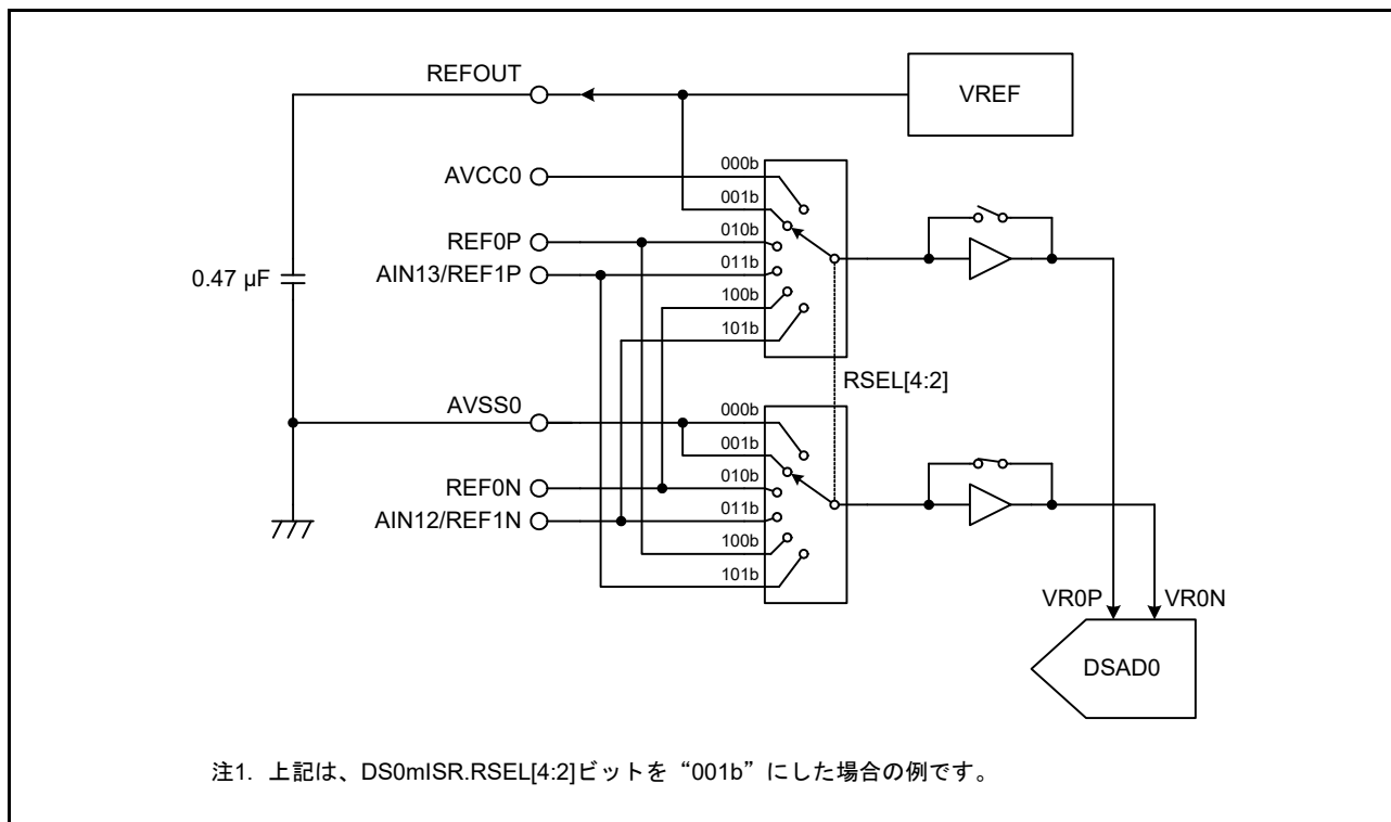
図 35.6 DSAD0 の + 側基準電圧に VREF の出力 (REFOUT) を使用する例
