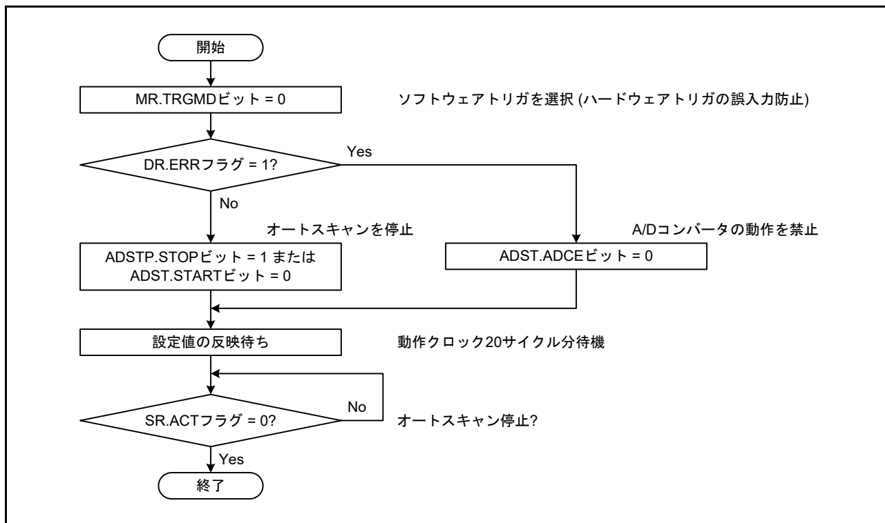
図 36.20 オートスキャン停止フロー
