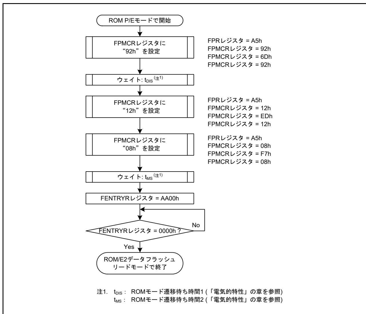
図 41.10 ROM P/E モードから ROM/E2 データフラッシュリードモードへの遷移フロー
