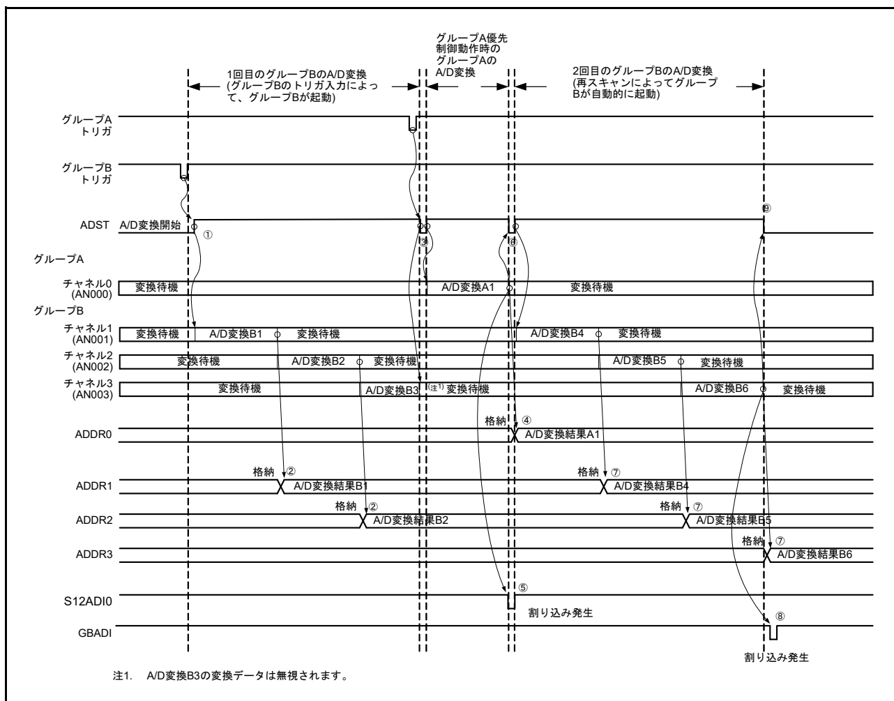
図 37.13 グループ A 優先制御の動作例 (1) (ADGSPCR.GBRSCN = 1、ADGSPCR.GBRP = 0 時の動作)
