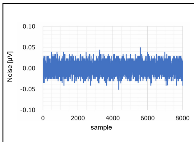
図 42.64 ノイズプロット (AVCC0 = 5.0V、 T_a = 25^\circ\text{C} 、Gain = 64、 f_{\text{MOD}} = 4\text{MHz} 、 f_{\text{DR}} = 3.8\text{ SPS} 、Sinc 4 +Sinc 4 フィルタ、 V_{\text{ID}} = 0\text{V} 、 V_{\text{REF}} = 2.5\text{V} 、リファレンスバッファ無効)
