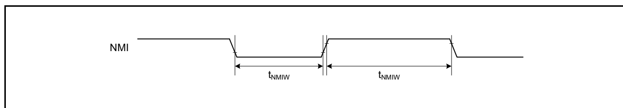
図 42.29 NMI 割り込み入力タイミング
