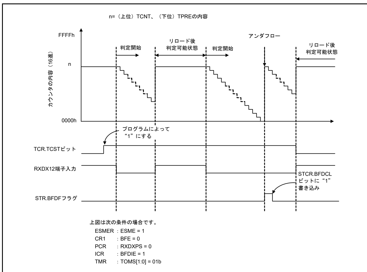
図 29.74 Break Field Low width 判定モードの動作例
