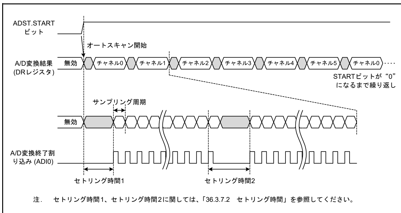
図 36.6 オートスキャンシーケンス
