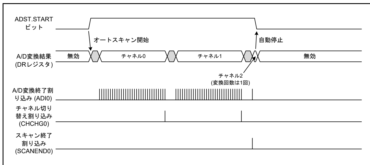
図 36.8 ワンショット動作
