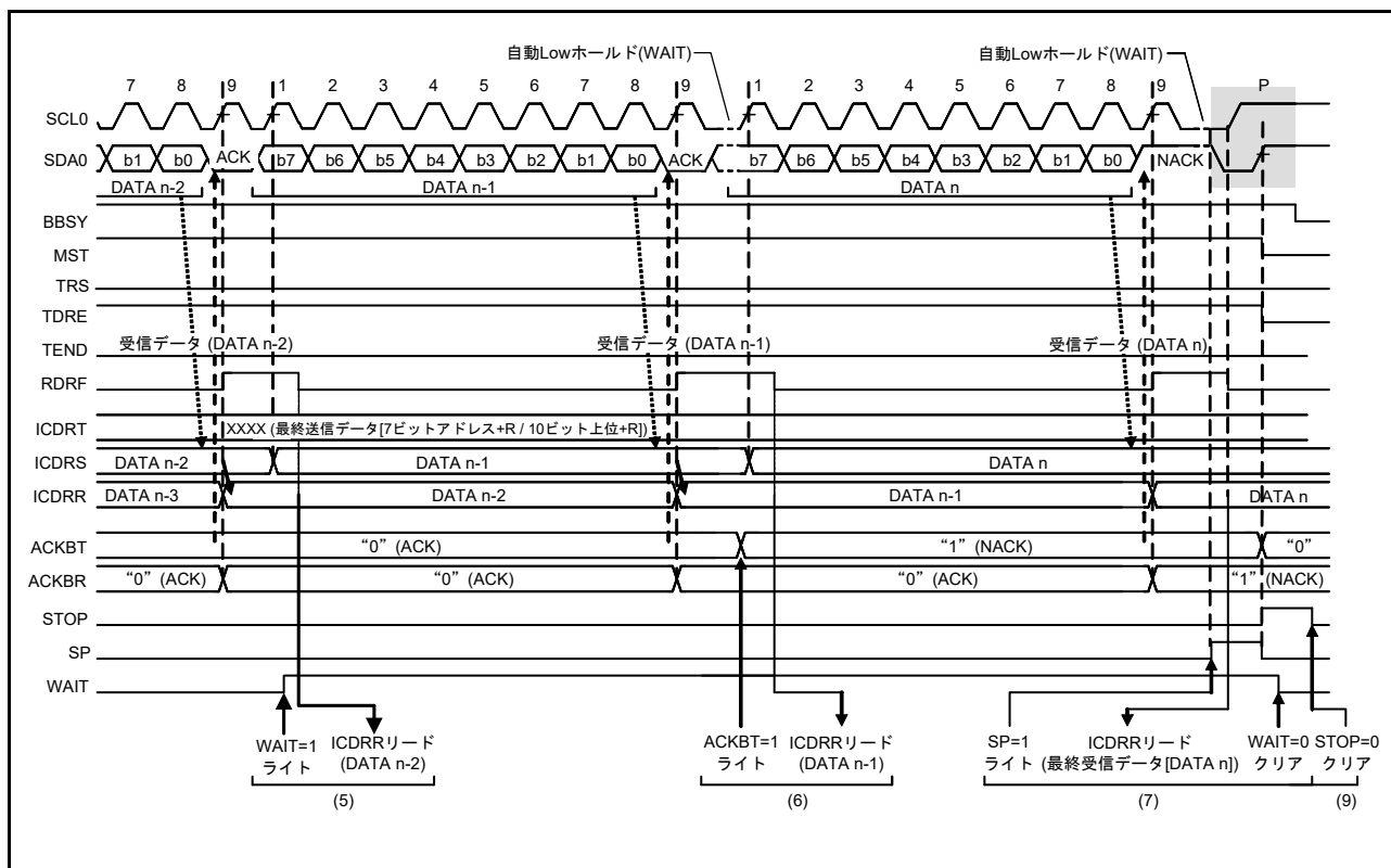
図 30.13 マスタ受信の動作タイミング (3) (RDRFS ビット = 0 のとき)
