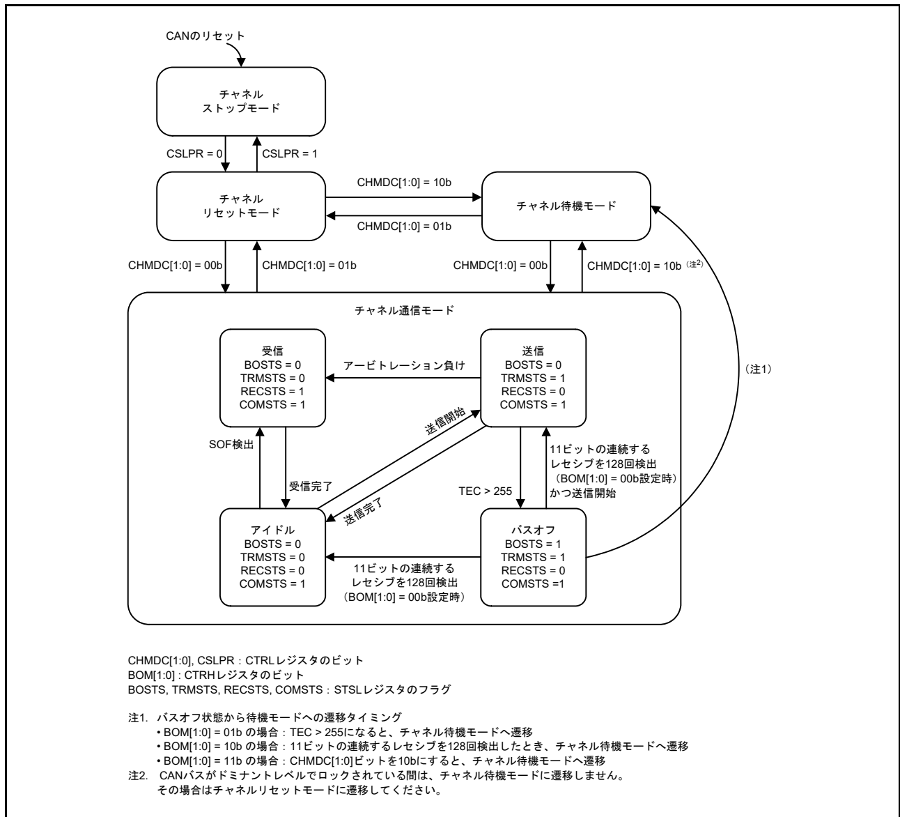
図 31.3 チャネルモードの状態遷移図
