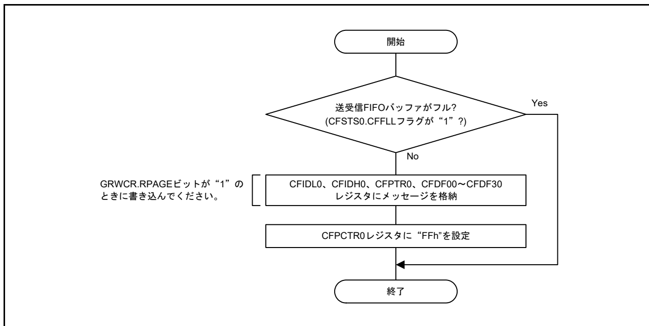
図 31.29 送受信 FIFO バッファからの送信手順
