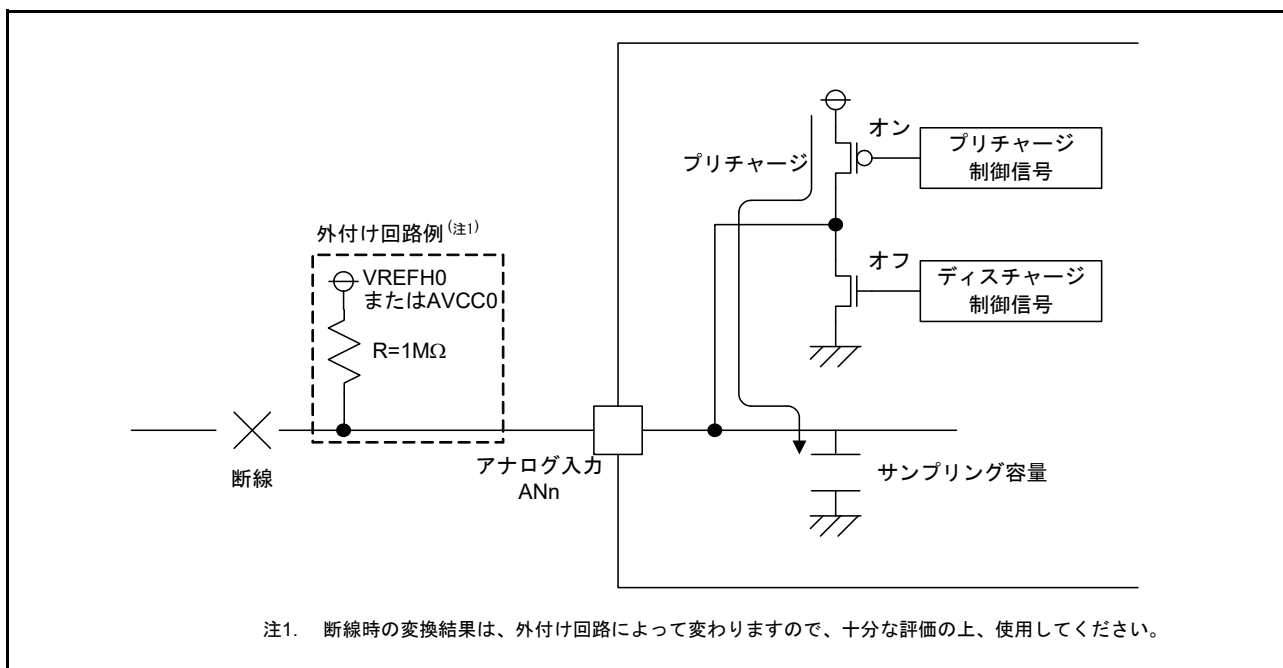
図 37.24 プリチャージを選択した場合の断線検出例
