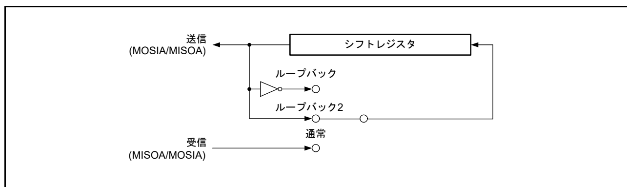
図 32.50 ループバックモード時のシフトレジスタ入出力構成 (マスターモード)
