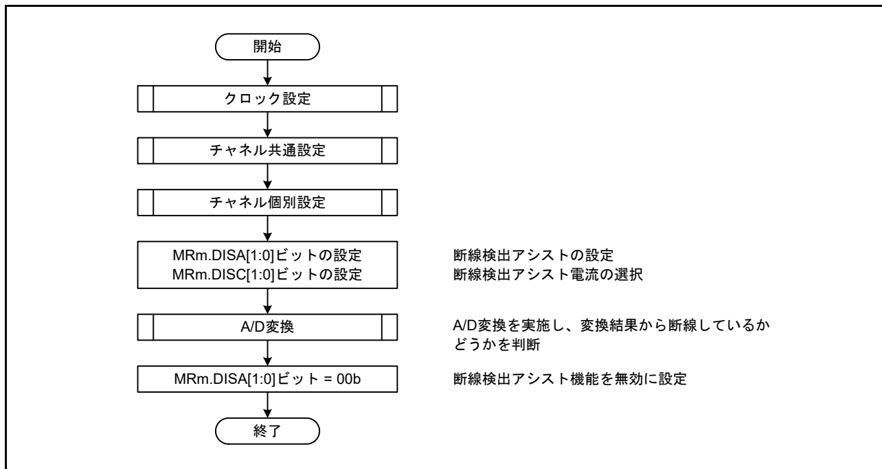
図 36.22 断線検出フロー (m = 0 ~ 7)
