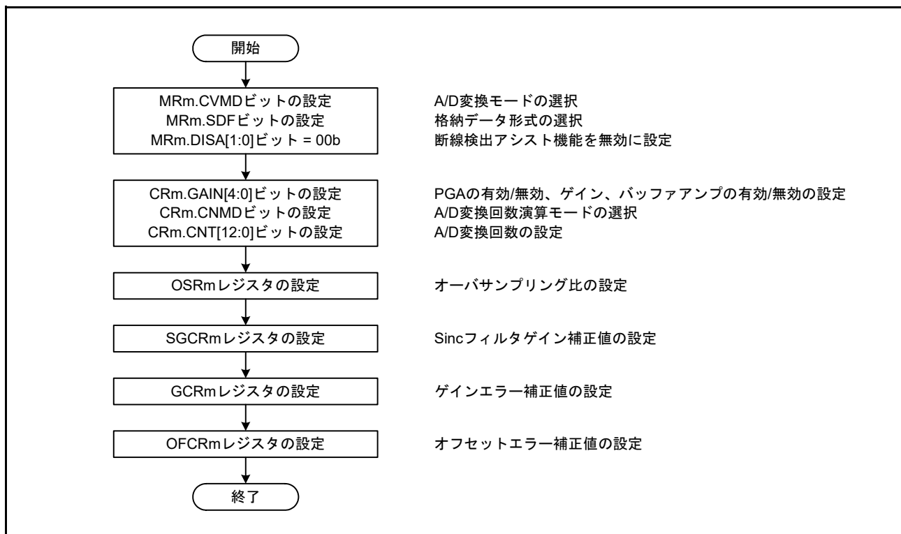
図 36.18 チャネル個別設定フロー (m = 0 ~ 7)
