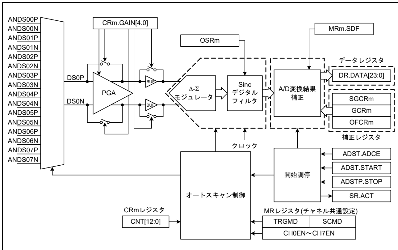
図 36.4 DSAD のブロック図 (m = 0 ~ 7)
