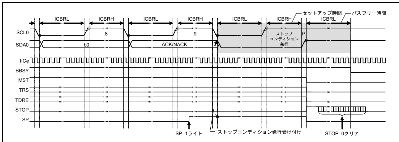
図 30.37 ストップコンディション発行動作タイミング (SP ビット)
