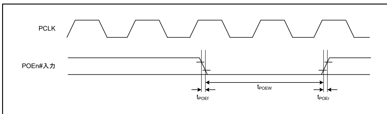
図 42.34 POE 入力タイミング (n = 0 ~ 3, 8)
