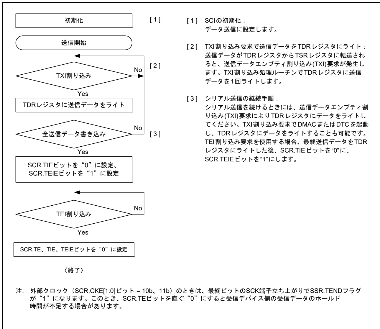
図 29.28 クロック同期式モードのシリアル送信のフローチャート例
