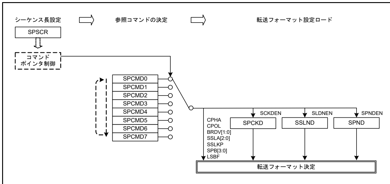
図 32.45 マスタモードでのシリアル転送方式の決定方法
