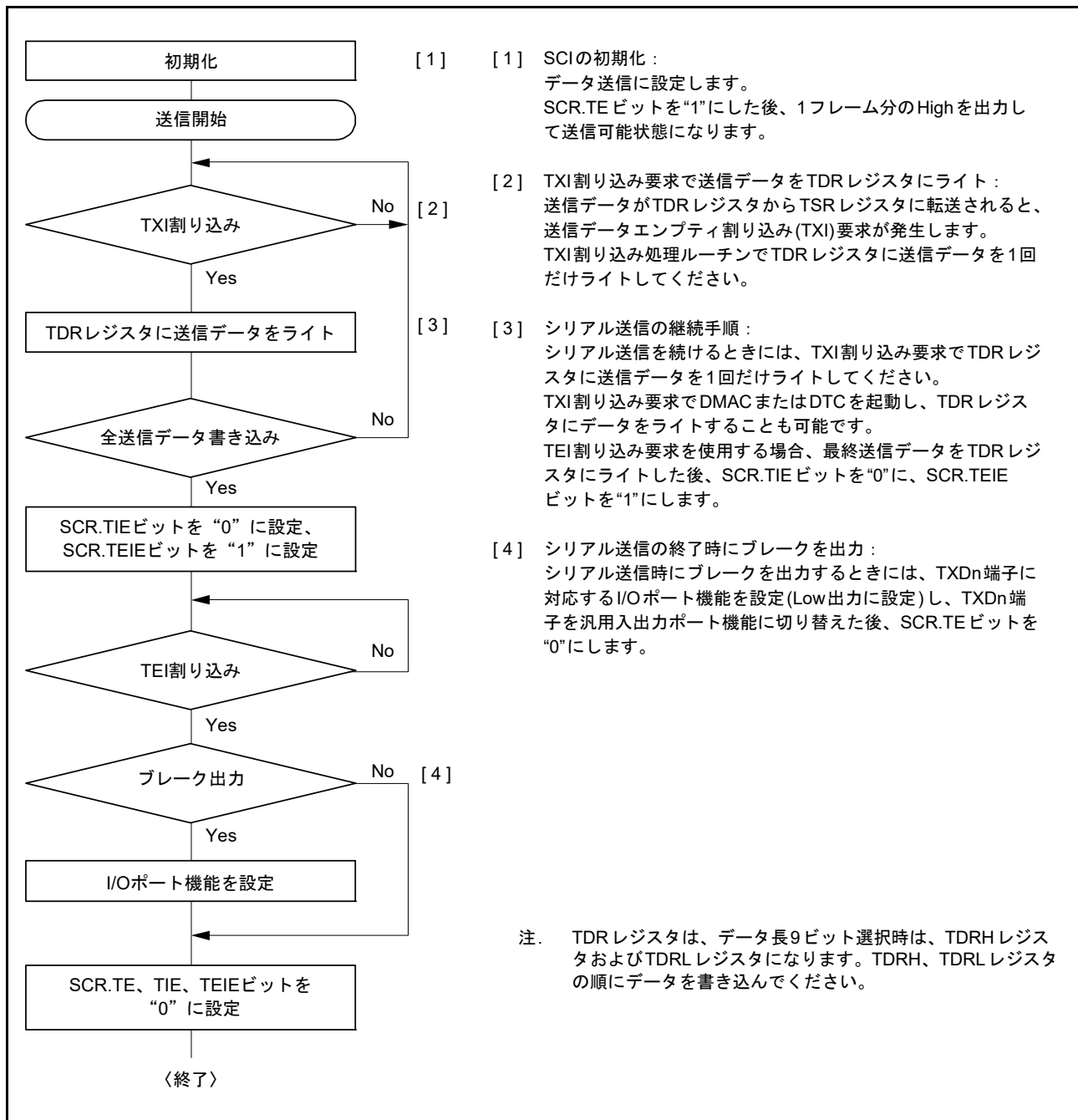
図 29.13 調歩同期式モードのシリアル送信のフローチャート例
