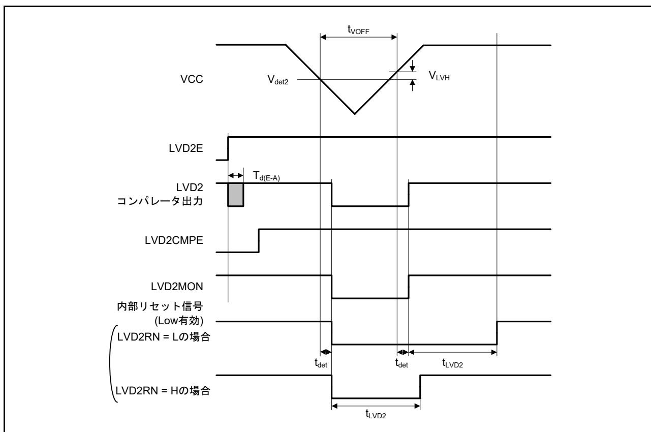
図 42.55 電圧検出回路タイミング (V det2 )
