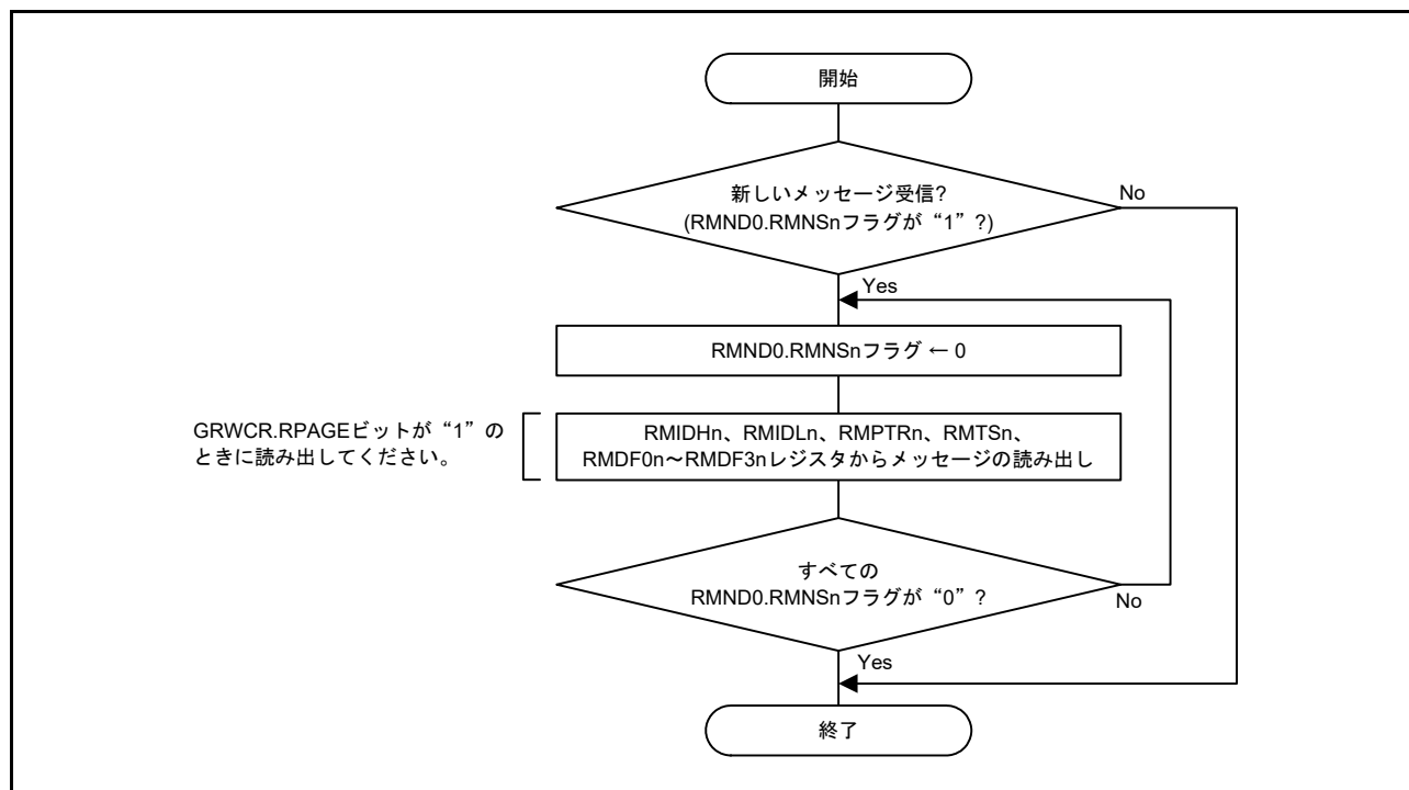
図 31.22 受信バッファの読み出し手順
