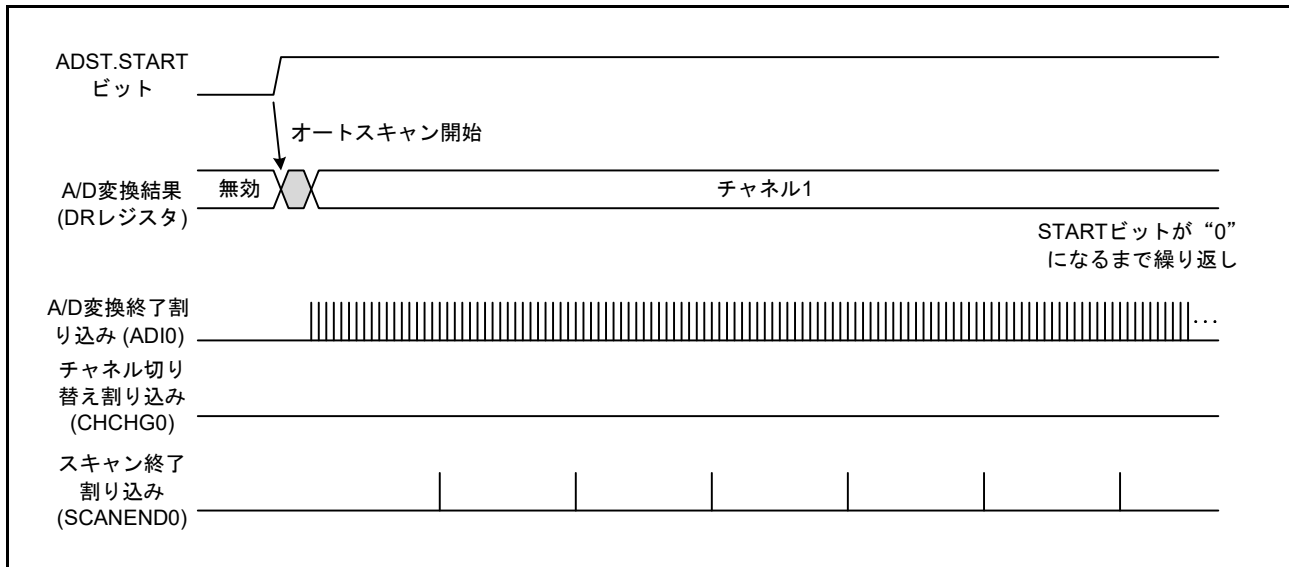
図 36.9 単一チャンネルの連続変換
