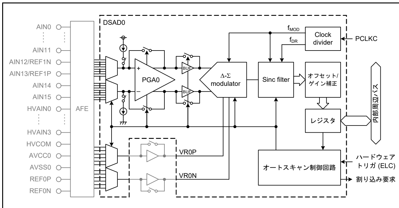
図 36.1 DSADのブロック図
