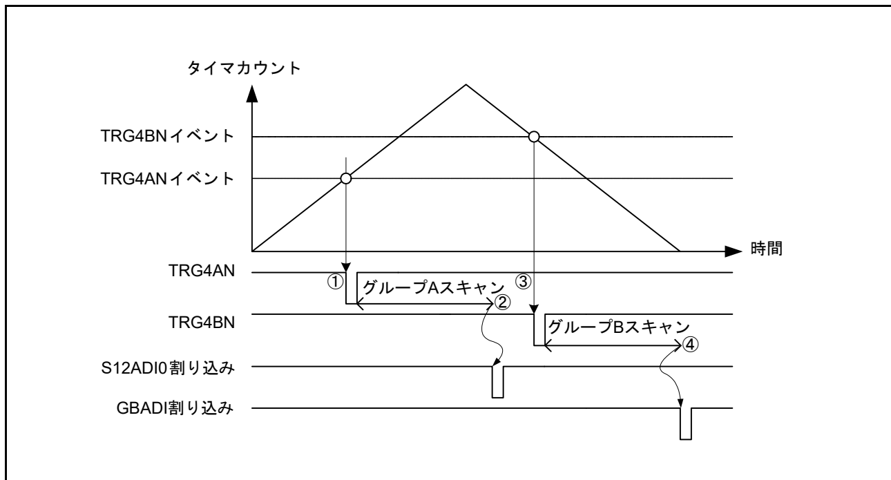
図 37.10 グループスキャンモードの動作例 (MTU からの同期トリガ発生による基本動作)
