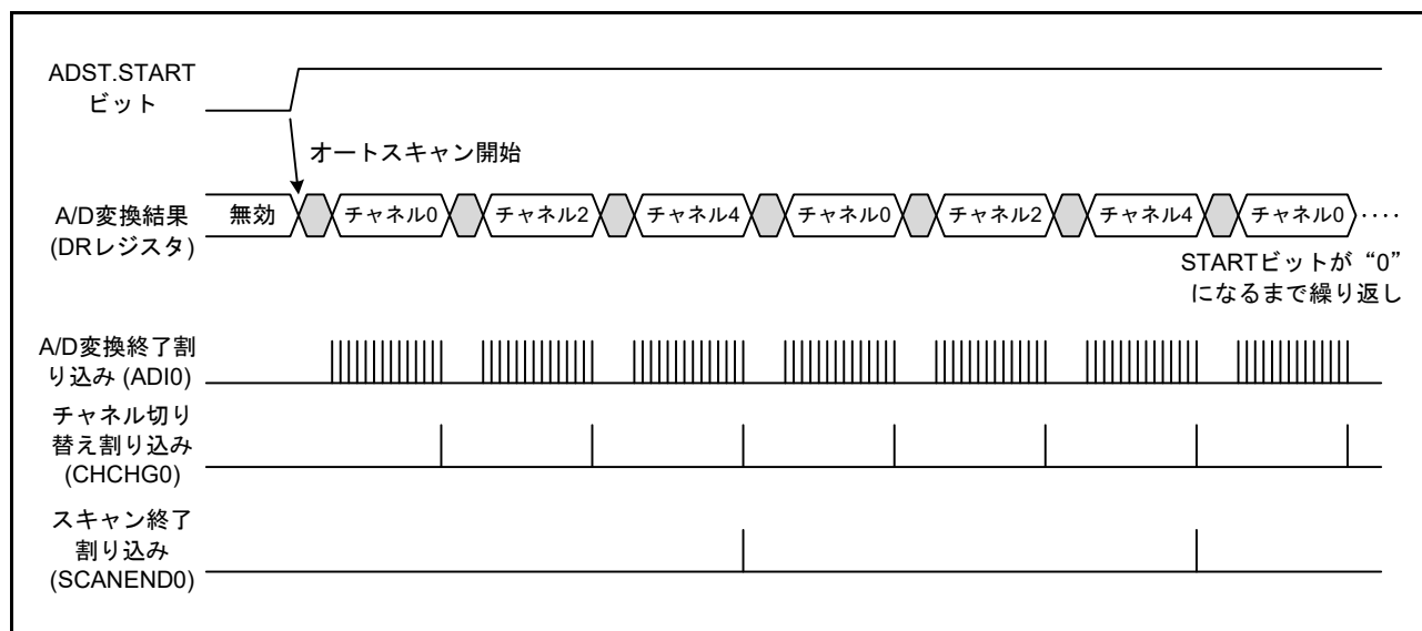
図 36.7 変換チャンネルのスキップ
