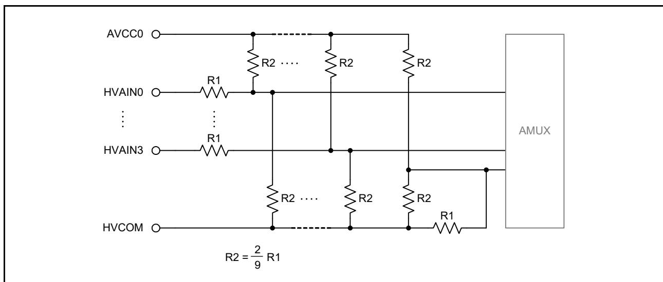
図 35.5 HVAC のブロック図
