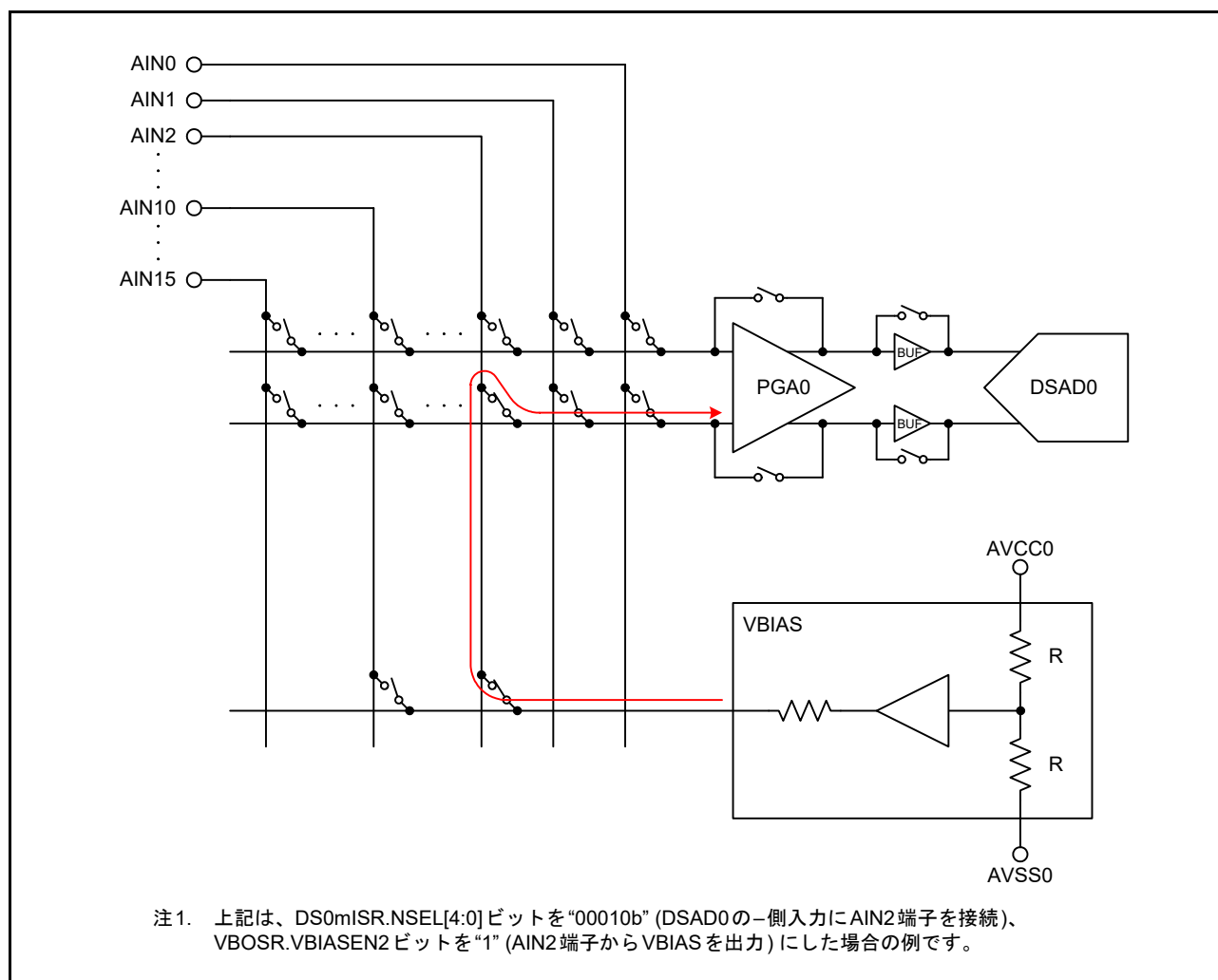
図 35.7 VBIAS と PGA の接続例
