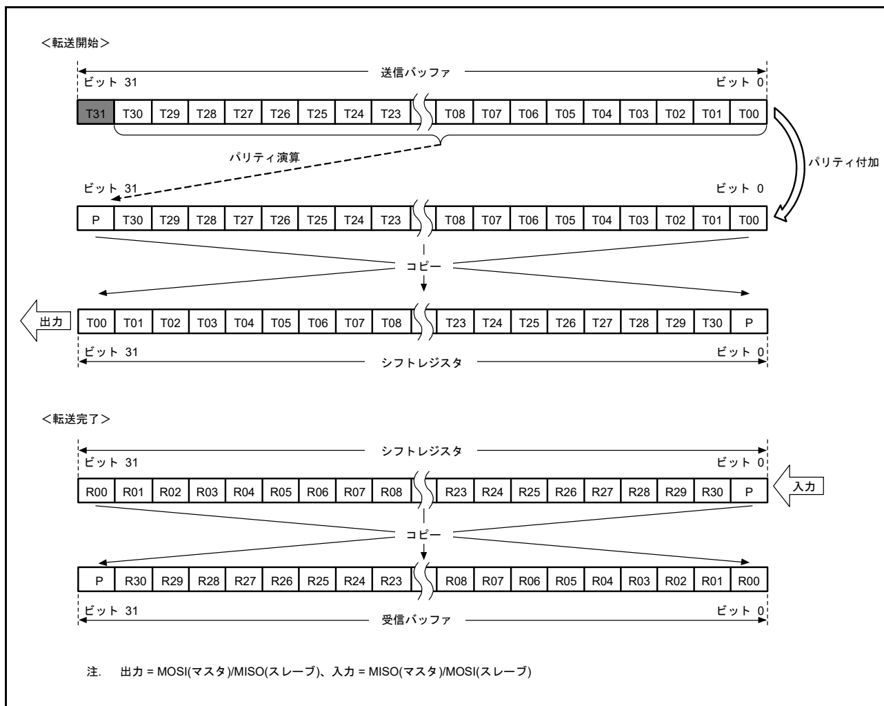
図 32.20 LSB ファースト転送 (32 ビットデータ / パリティ機能有効)
