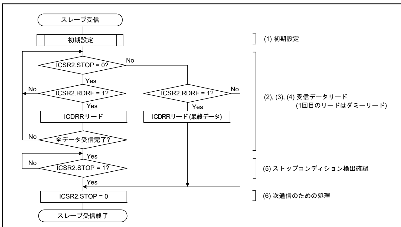
図 30.17 スレーブ受信のフローチャート例
