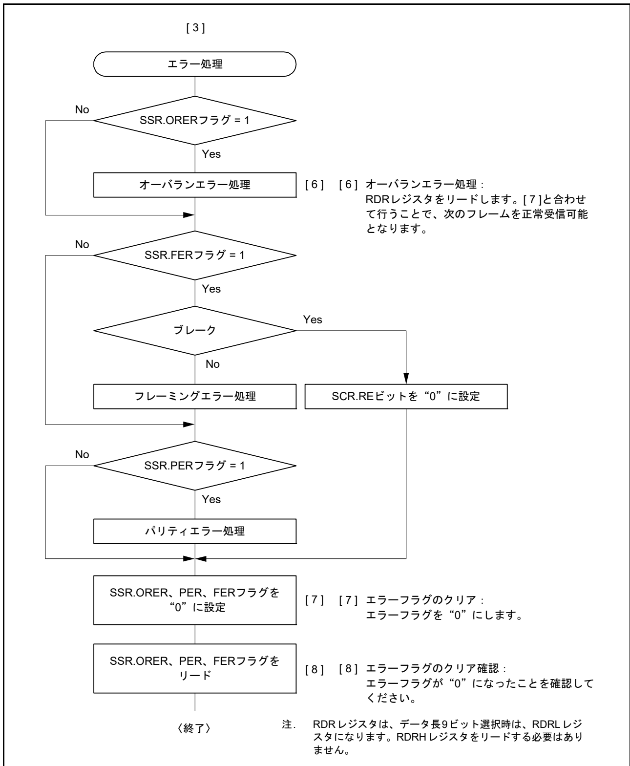
図 29.17 調歩同期式モードのシリアル受信のフローチャート例 (2)
