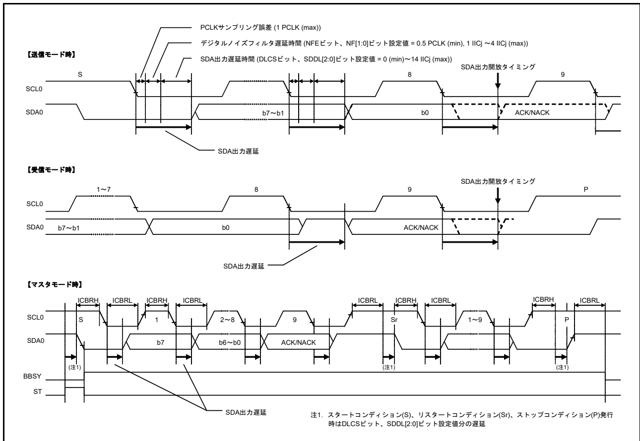
図 30.21 SDA出力遅延タイミング
