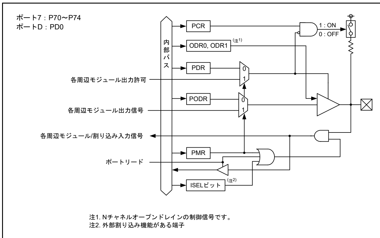
図 20.5 入出力ポートの構成 (5)
