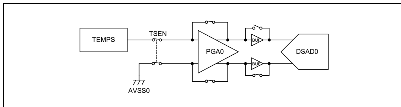
図 35.8 TEMPS の使用方法
