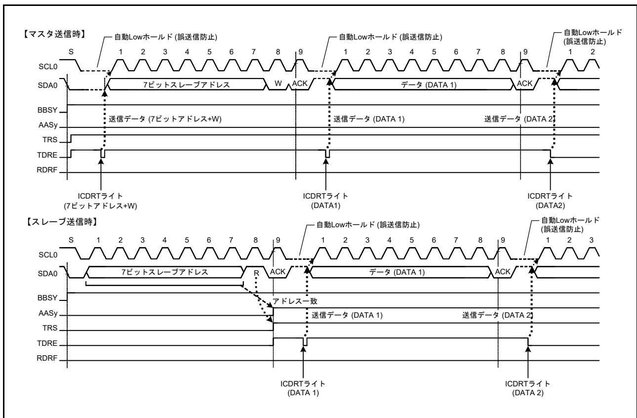
図 30.29 送信モードの自動Lowホールド動作
