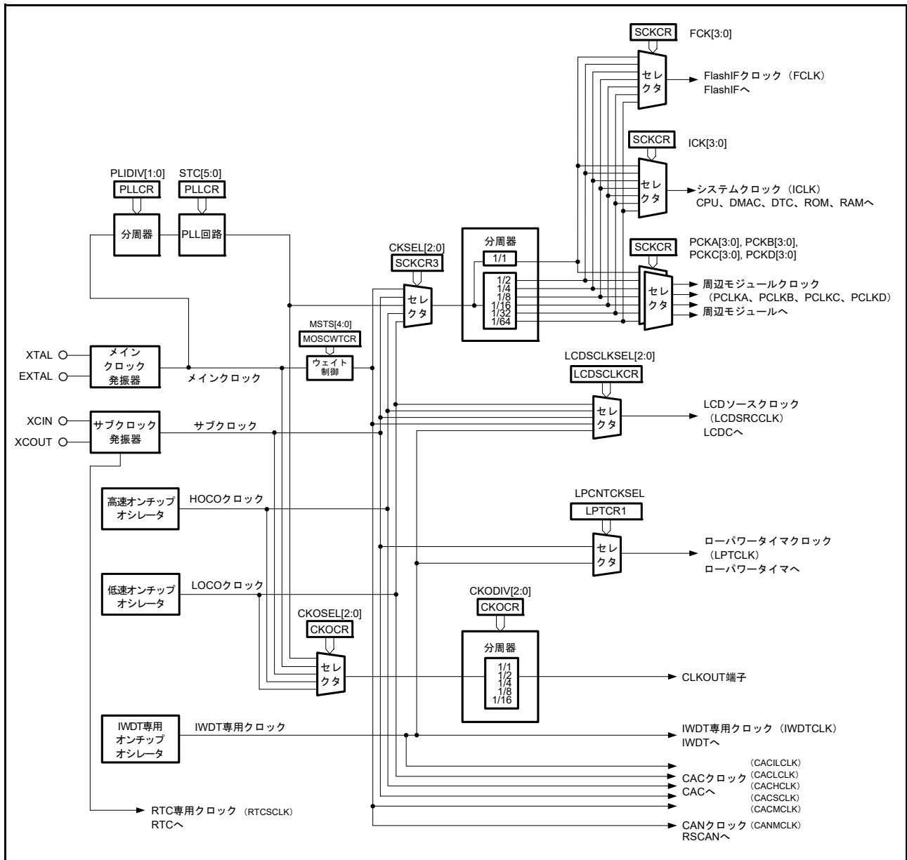
図 9.1 クロック発生回路のブロック図
