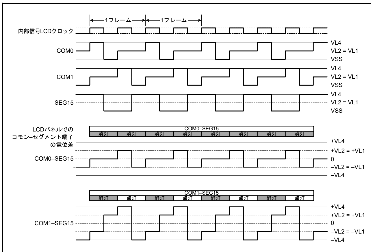
図 34.23 SEG15 端子と各コモン端子間の 1/2 デューティ LCD 駆動波形例 (1/2 バイアス)
