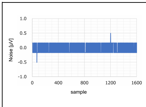
図 42.62 ノイズプロット (AVCC0 = 5.0V、 T_a = 25^\circ\text{C} 、Gain = 1 (PGA 無効、BUF 無効)、 f_{\text{MOD}} = 4\text{MHz} 、 f_{\text{DR}} = 3.8\text{ SPS} 、Sinc 4 +Sinc 4 フィルタ、 V_{\text{ID}} = 0\text{V} 、 V_{\text{REF}} = 2.5\text{V} 、リファレンスバッファ無効)
