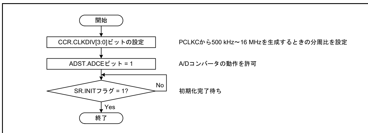
図 36.16 DSAD 起動フロー
