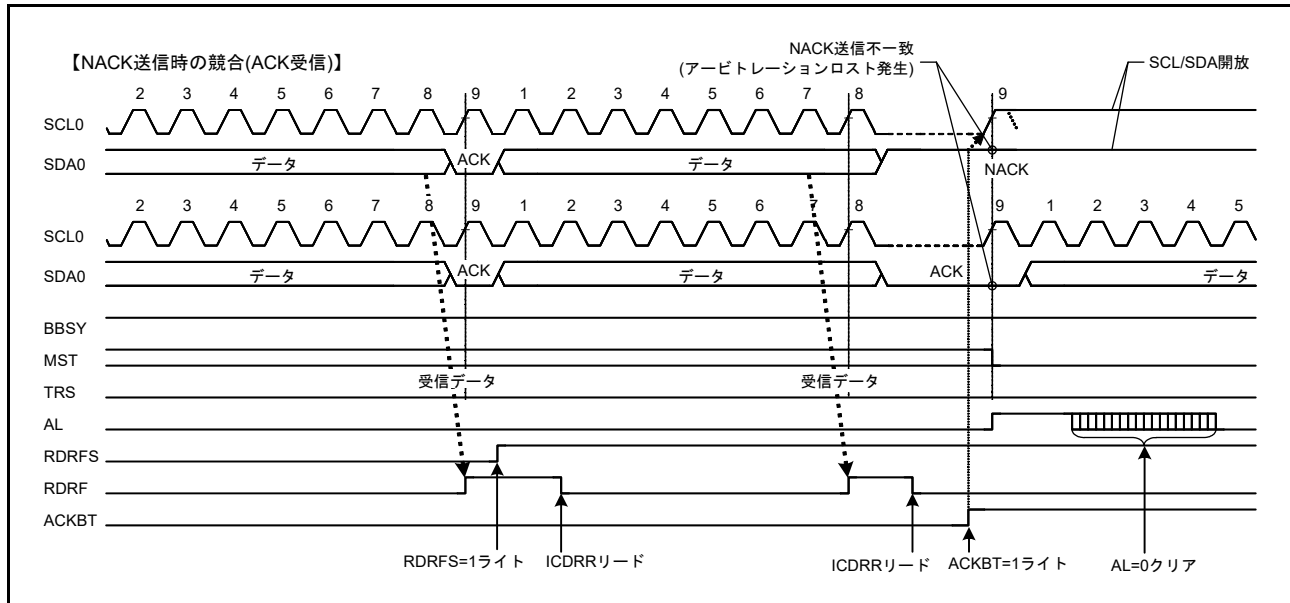
図 30.34 NACK 送信アービトレーションロスト検出動作例 (NALE ビット = 1 のとき)
