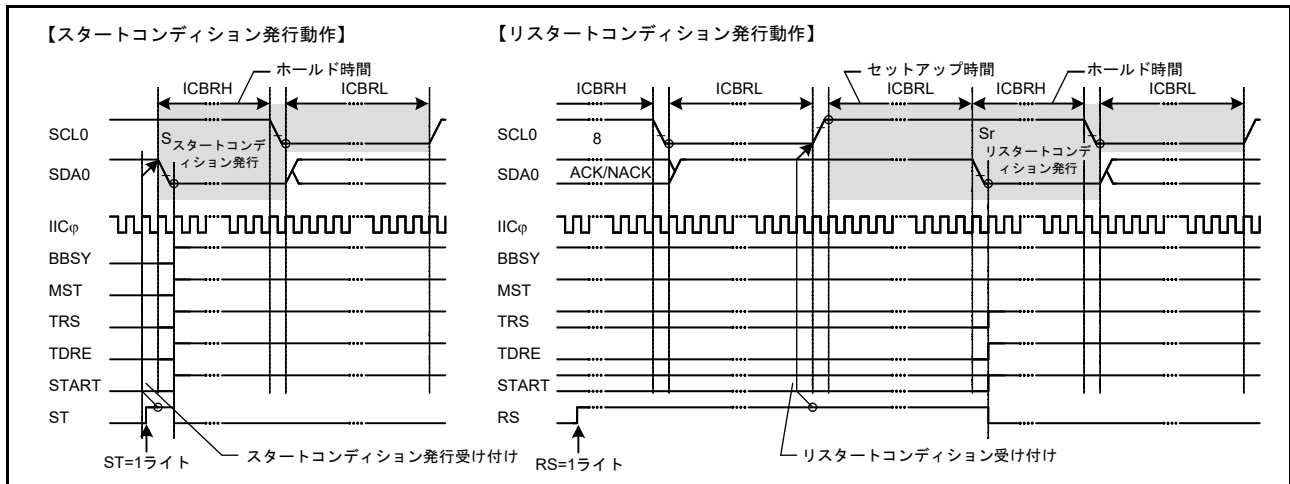
図 30.36 スタートコンディション/リスタートコンディション発行動作タイミング (ST、RS ビット)
