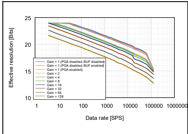
図 42.68 有効分解能のデータレート依存性 (AVCC0 = 5.0V、 T_a = 25^\circ\text{C} 、 f_{\text{MOD}} = 4\text{MHz} 、Sinc 4 フィルタまたは Sinc 4 +Sinc 4 フィルタ、 V_{\text{ID}} = 0\text{V} 、 V_{\text{REF}} = 2.5\text{V} 、リファレンスバッファ無効)
