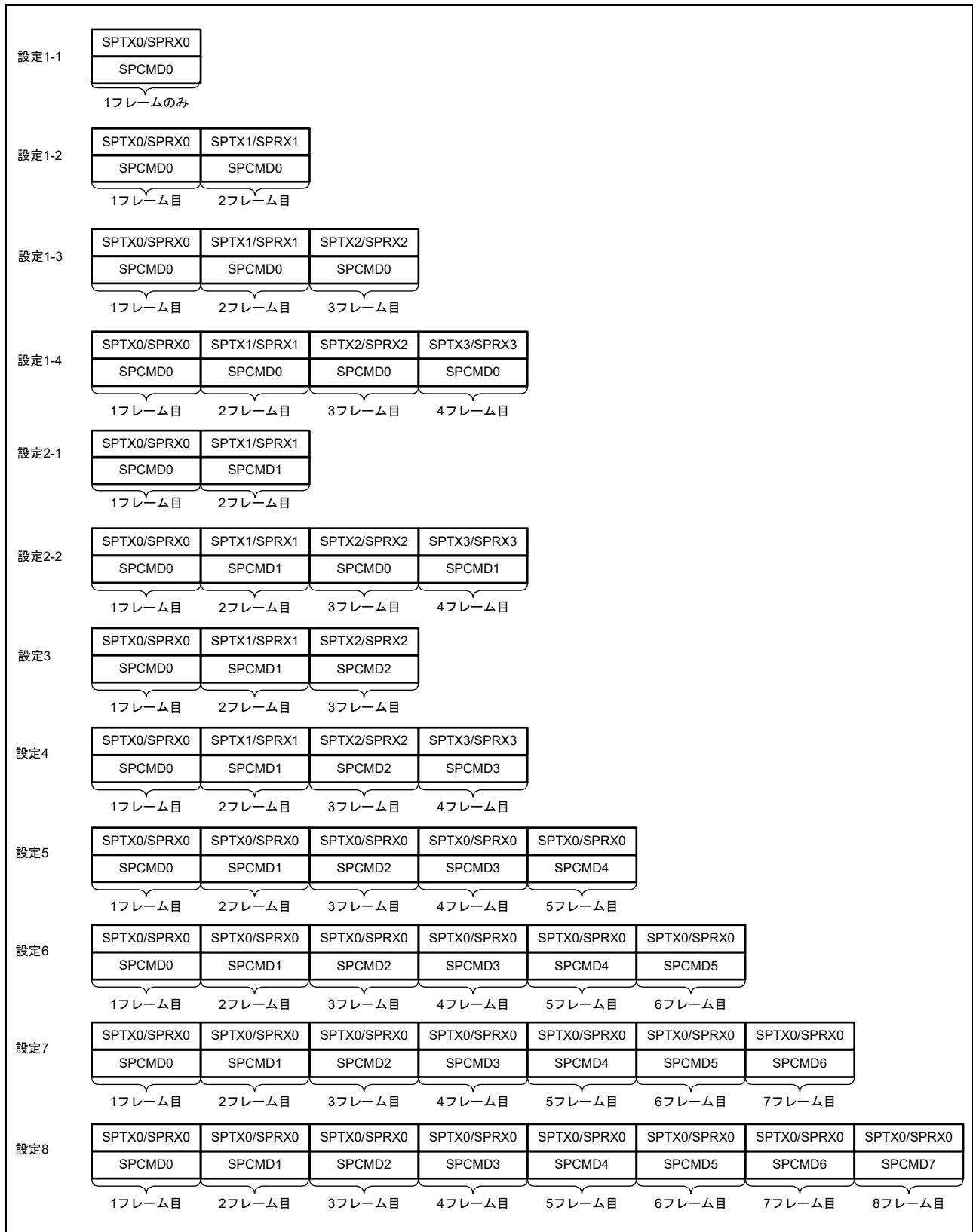
図 32.35 シーケンス動作時の RSPI コマンドレジスタと送受信バッファの対応
