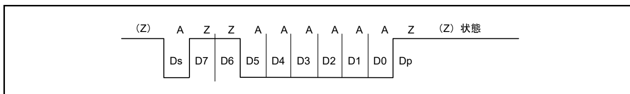
図 29.36 インバースコンベンション (SCMR.SDIR ビット = 1、SCMR.SINV ビット = 1、SMR.PM ビット = 1)
