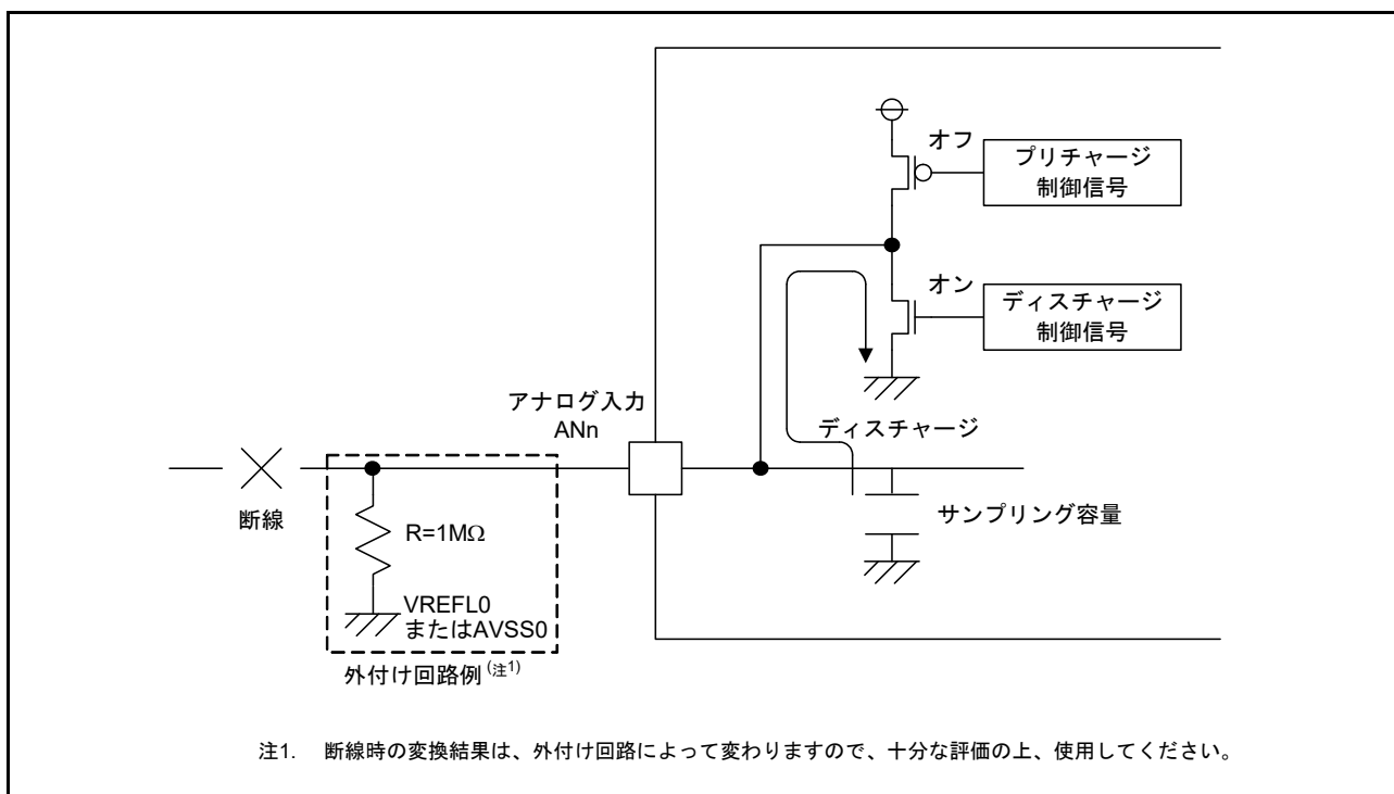
図 37.25 ディスチャージを選択した場合の断線検出例
