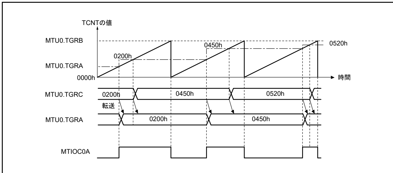
図 22.17 バッファ動作例 (1)
