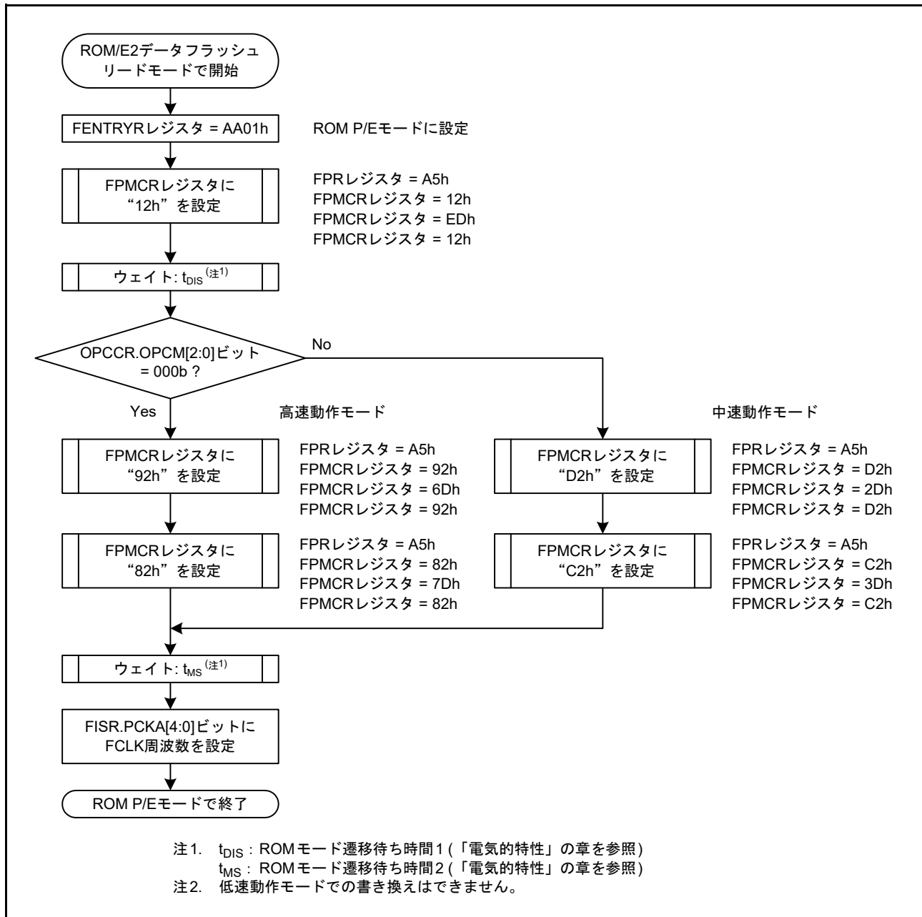
図 41.8 ROM/E2 データフラッシュリードモードから ROM P/E モードへの遷移フロー
