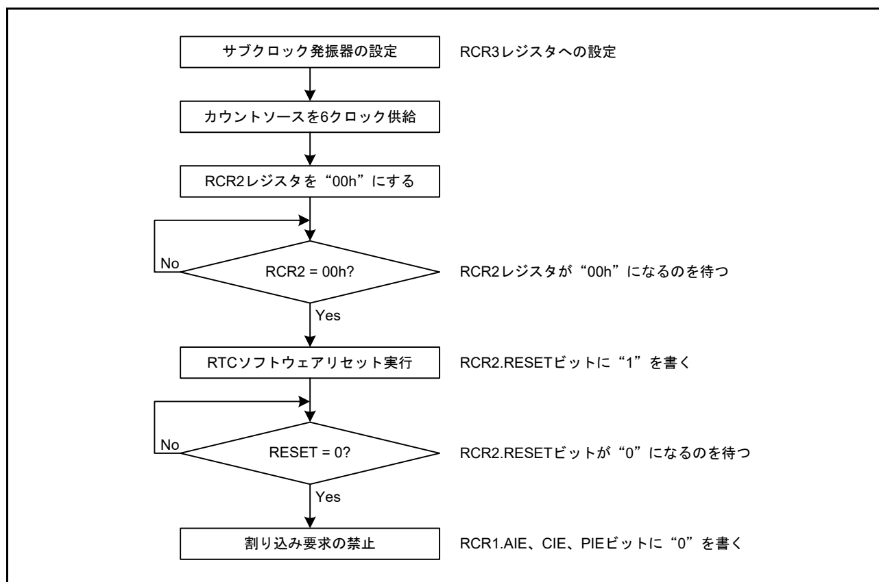
図 26.12 初期化手順
