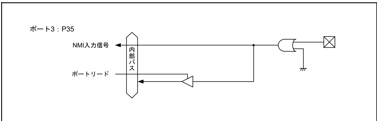
図 20.2 入出力ポートの構成 (2)
