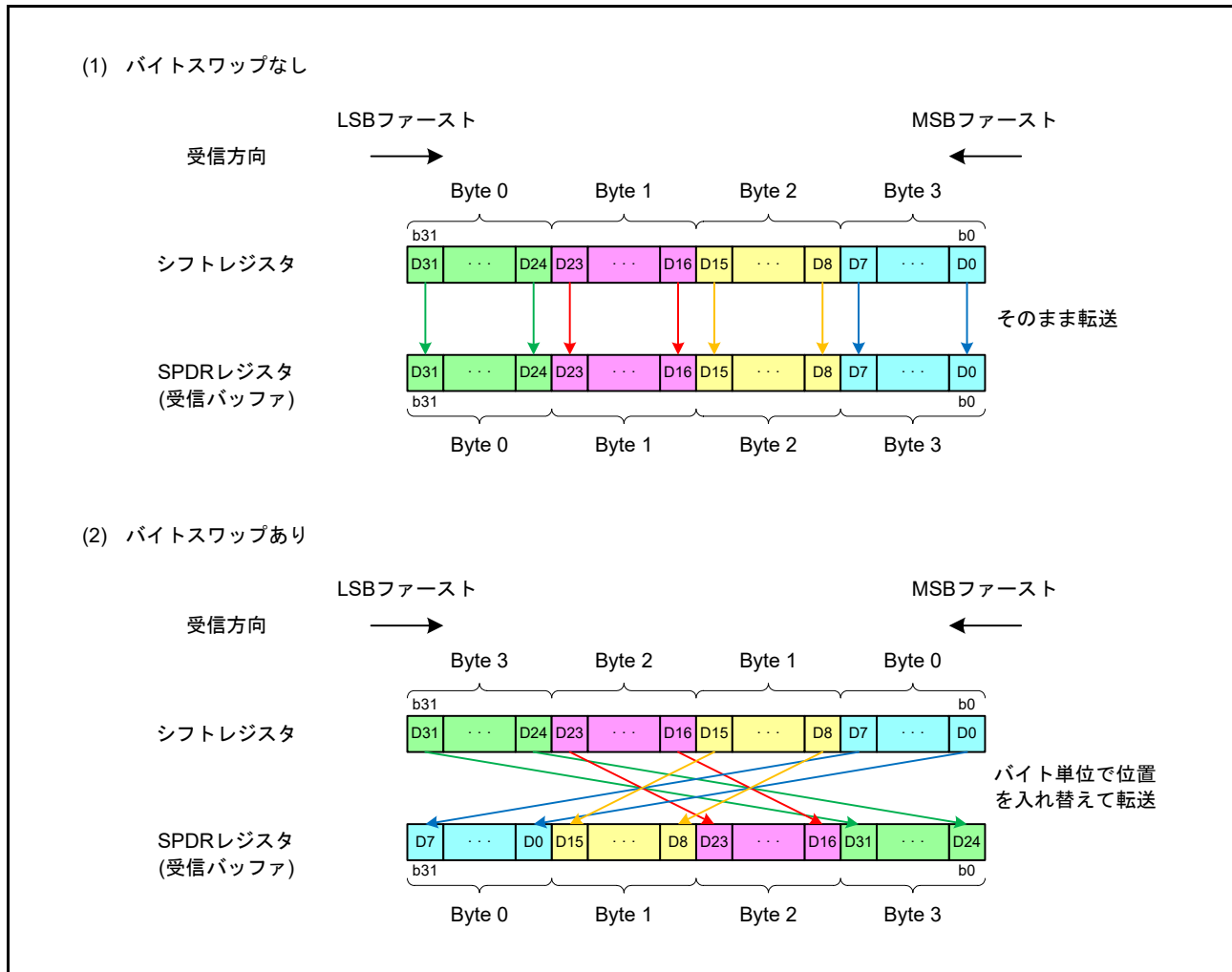
図 32.23 MSB/LSB ファーストとバイトスワップあり/なしの設定と受信データ変換
