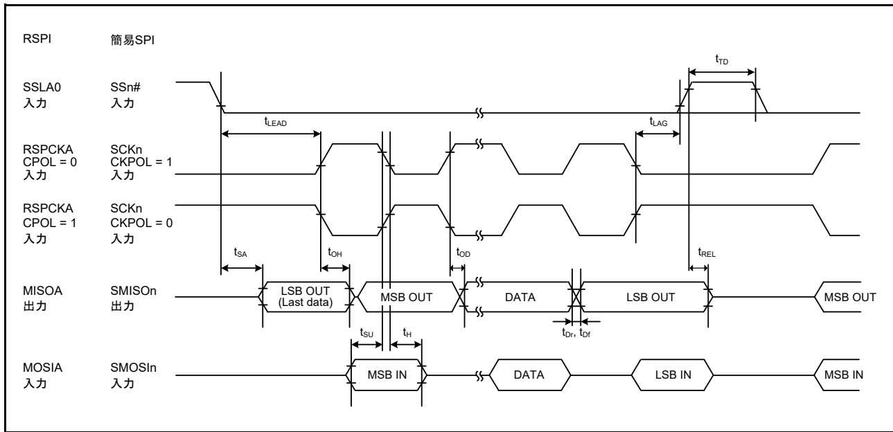
図 42.47 RSPI タイミング (スレーブ、CPHA = 1)/ 簡易 SPI クロックタイミング (スレーブ、CKPH = 0) (n = 0, 1, 5, 6, 8, 9, 12)
