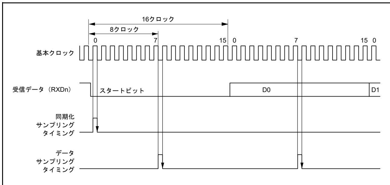
図 29.6 調歩同期式モードの受信データサンプリングタイミング
