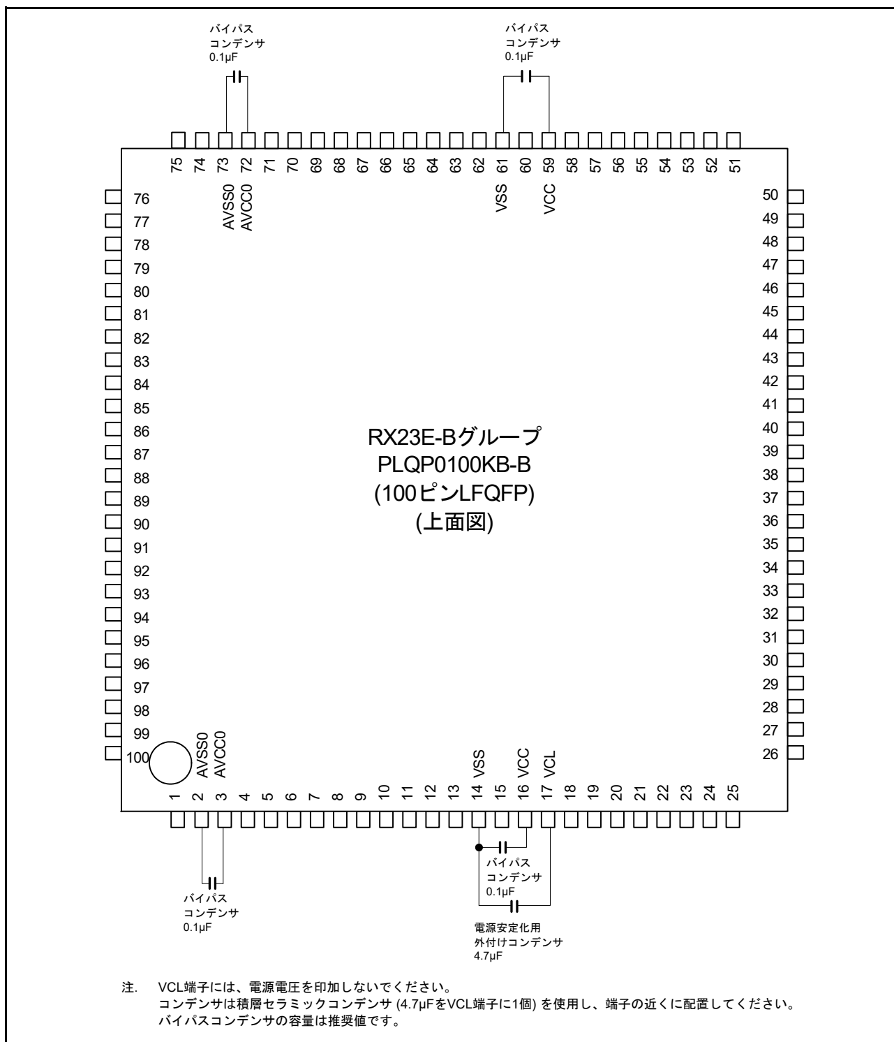
図 42.101 コンデンサ接続方法 (100ピン)
