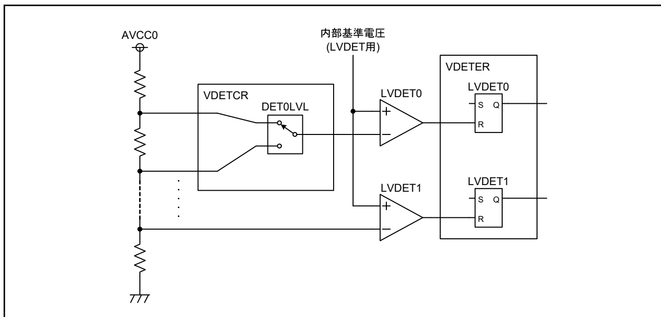
図 35.10 LVDET のブロック図
