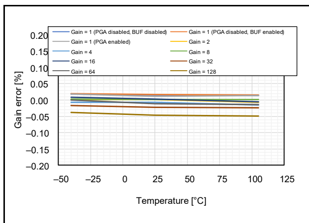
図 42.71 ゲイン誤差の温度依存性 (AVCC0 = 5.0V、 f_{\text{MOD}} = 4\text{MHz} 、総合 OSR = 4096、 V_{\text{REF}} = 2.5\text{V} )
