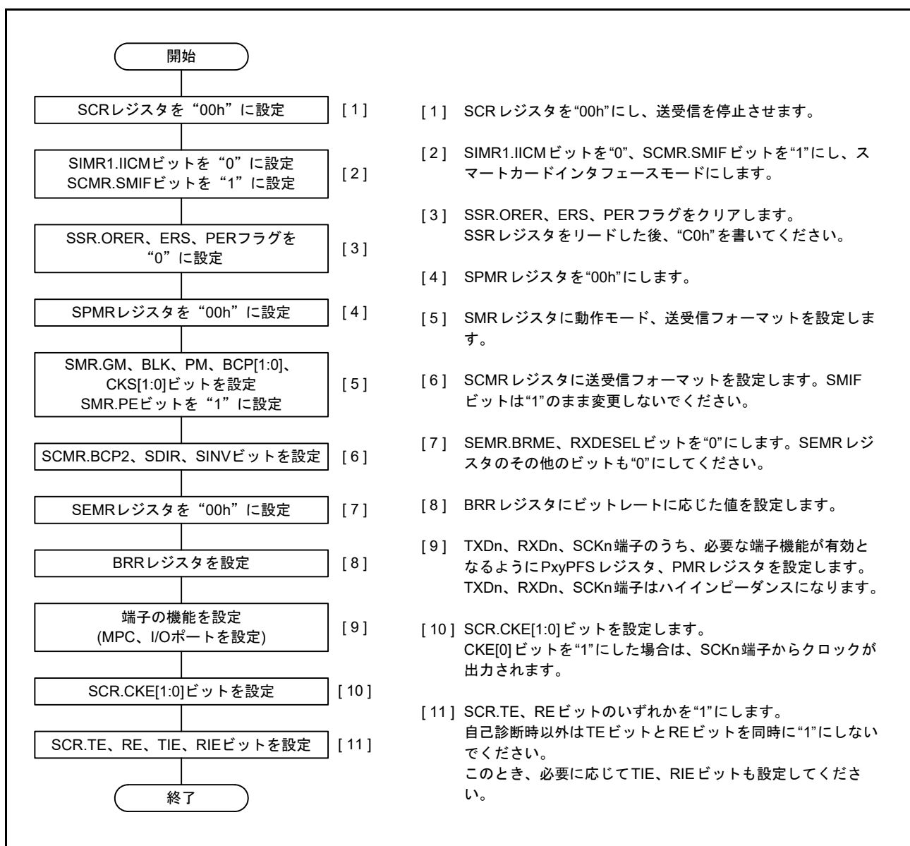
図 29.38 SCIの初期化フローチャートの例(スマートカードインタフェースモード)
