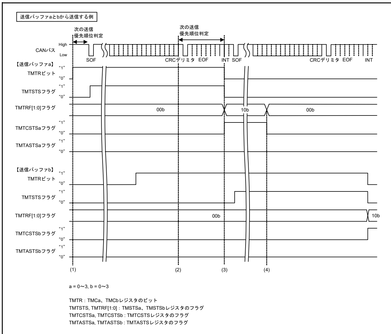
図 31.27 送信バッファの送信タイミング図 (正常に送信完了時)
