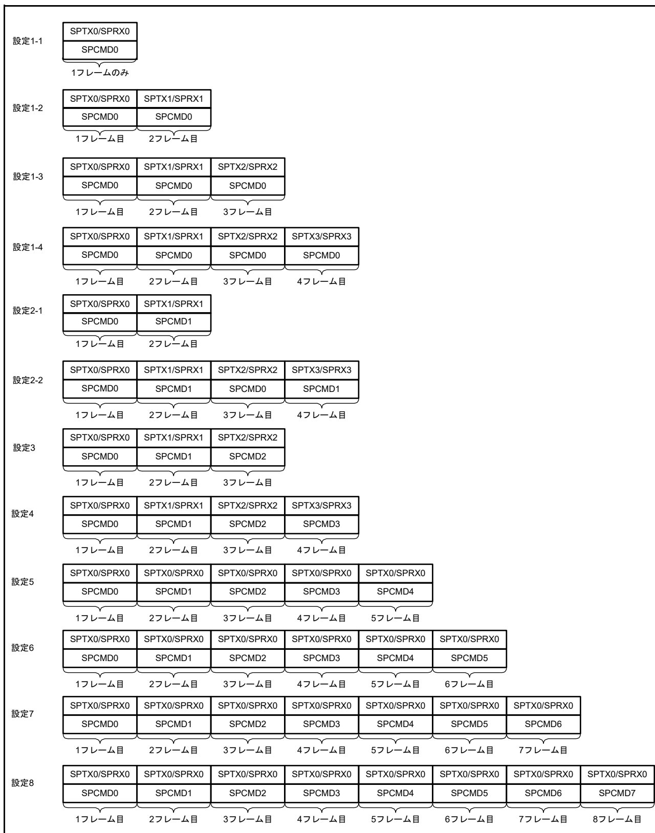
図 32.47 シーケンス動作時の RSPI コマンドレジスタと送受信バッファの対応
