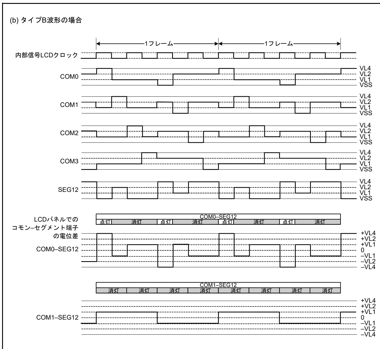
図 34.31 SEG12 端子と各コモン端子間の 1/4 デューティ LCD 駆動波形例 (1/3 バイアス) (2)
