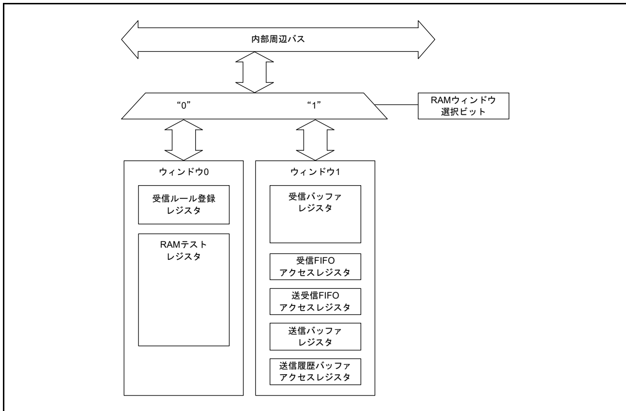
図 31.15 RAM ウィンドウ
