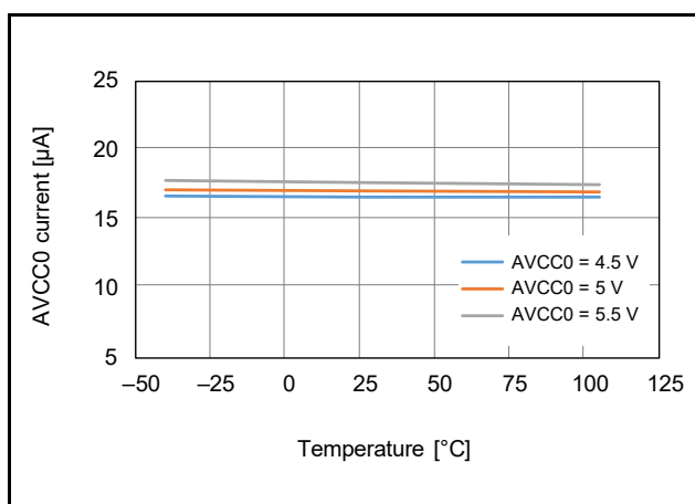
図 42.11 バイアス電圧生成回路動作電流の温度依存性
