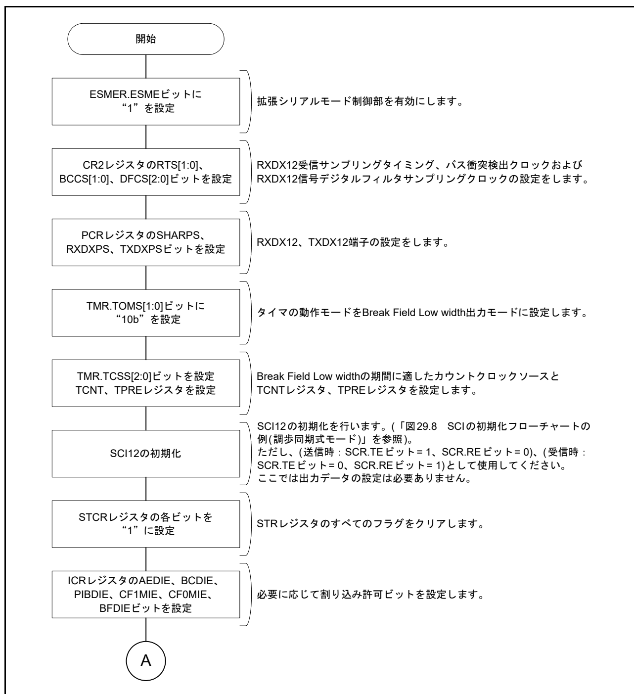
図 29.62 Start Frame 送信フローチャート例 (1)
