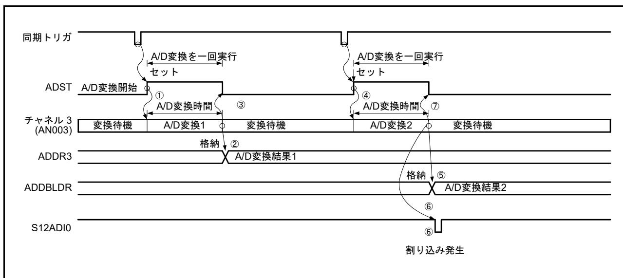
図 37.7 シングルスキャンモードの動作例 (ダブルトリガモード選択、AN003を二重化)
