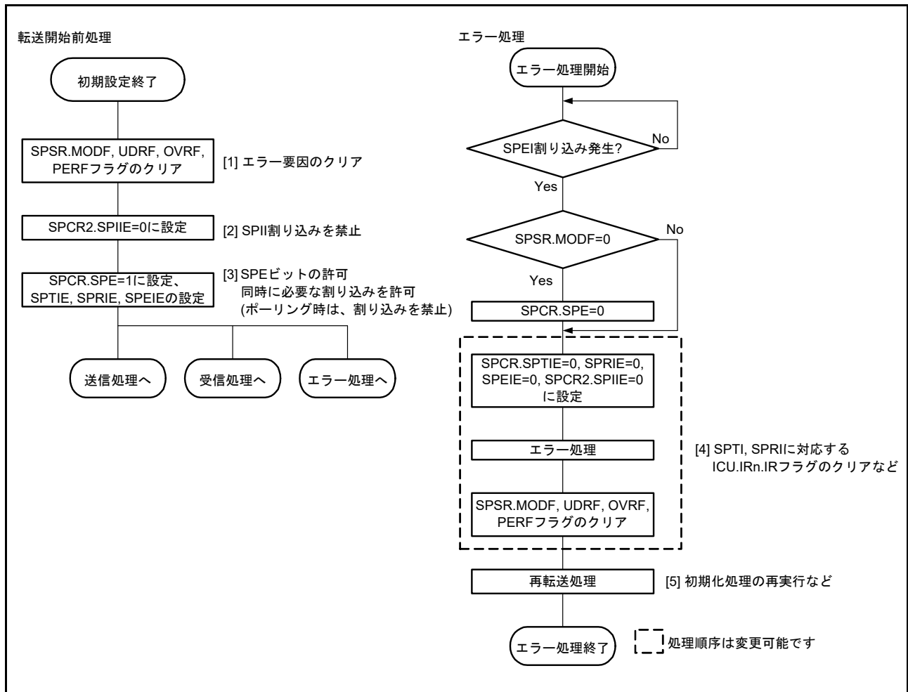
図 32.44 スレーブモード時のフローチャート (エラー処理)
