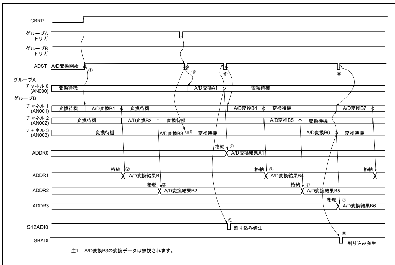
図 37.17 グループ A 優先制御の動作例 (5) (ADGSPCR.GBRP = 1 時の動作)
