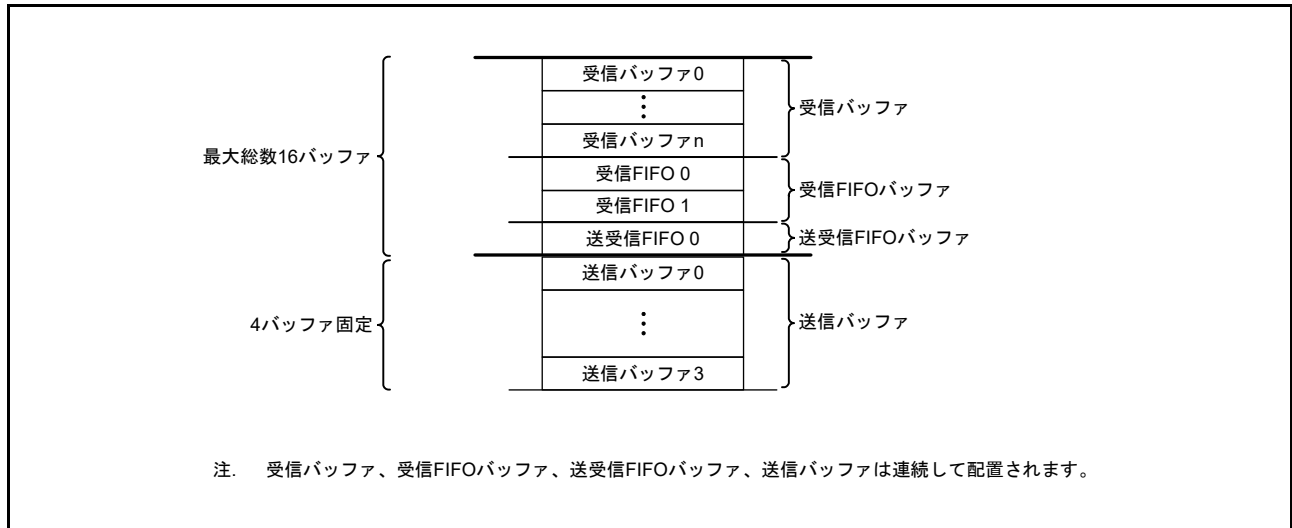
図 31.20 バッファの構成
