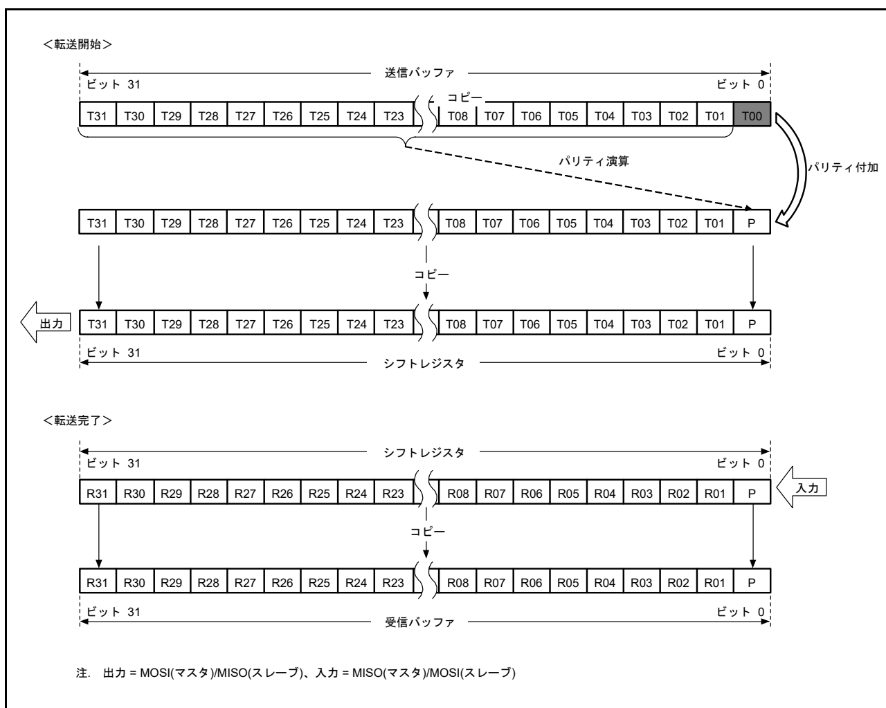
図 32.18 MSB ファースト転送 (32 ビットデータ / パリティ機能有効)
