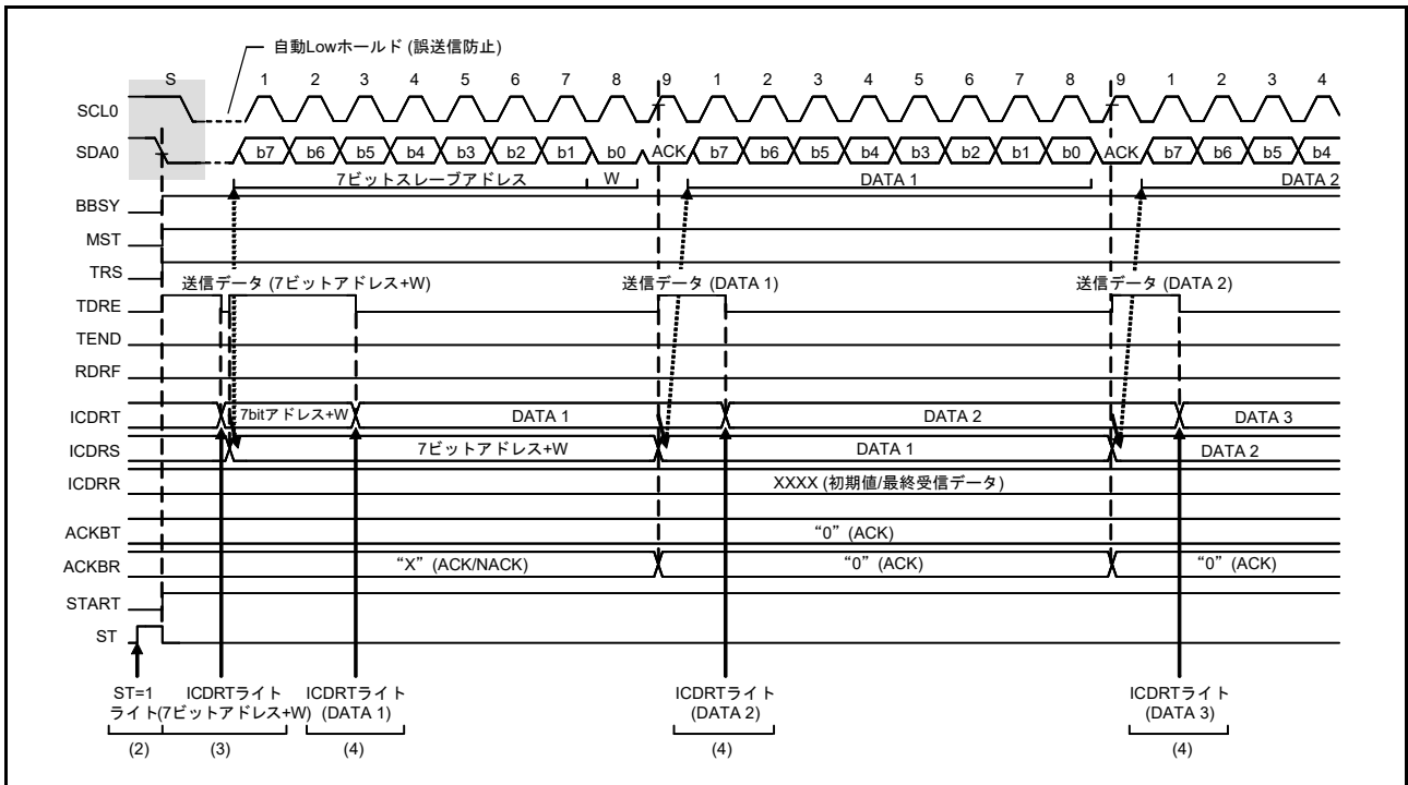
図 30.6 マスタ送信の動作タイミング (1) (7ビットアドレスフォーマットのとき)
