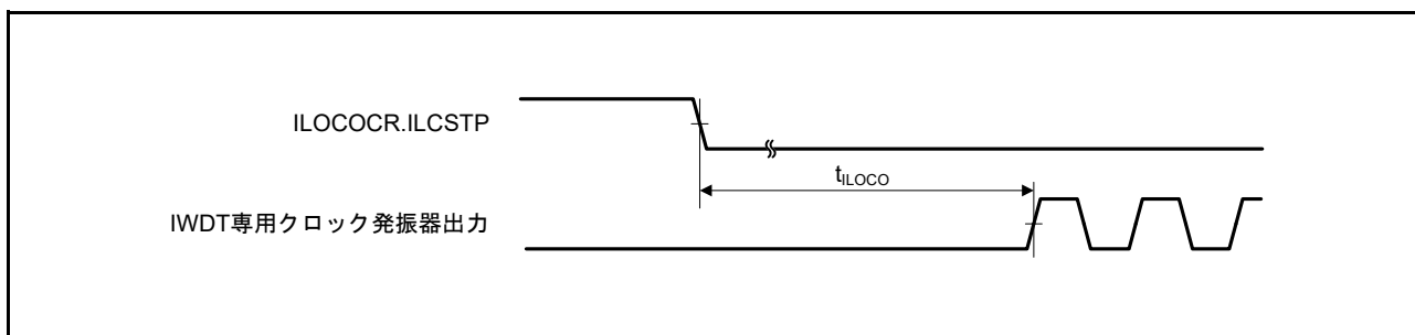
図 42.19 IWDW 専用クロック発振開始タイミング
