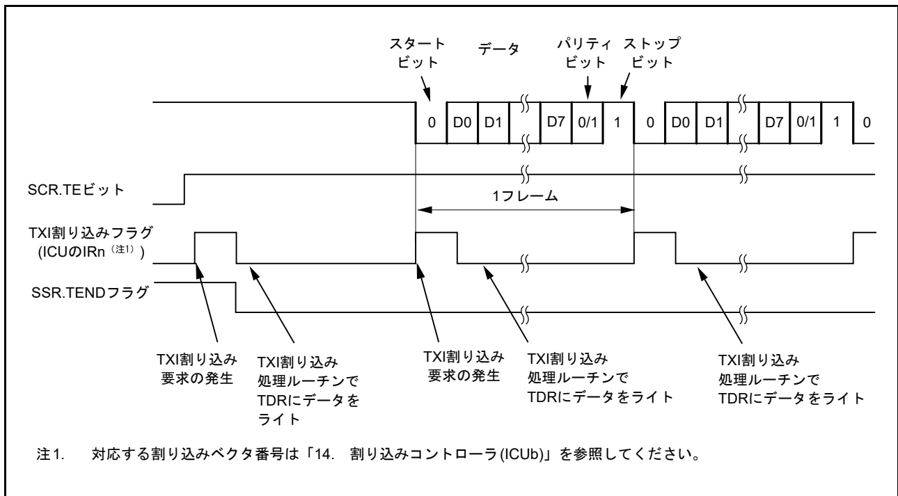
図 29.10 調歩同期式モードのシリアル送信の動作例 (1) (8ビットデータ / パリティあり / 1ストップビット / CTS 機能使用しない / 送信開始時)
