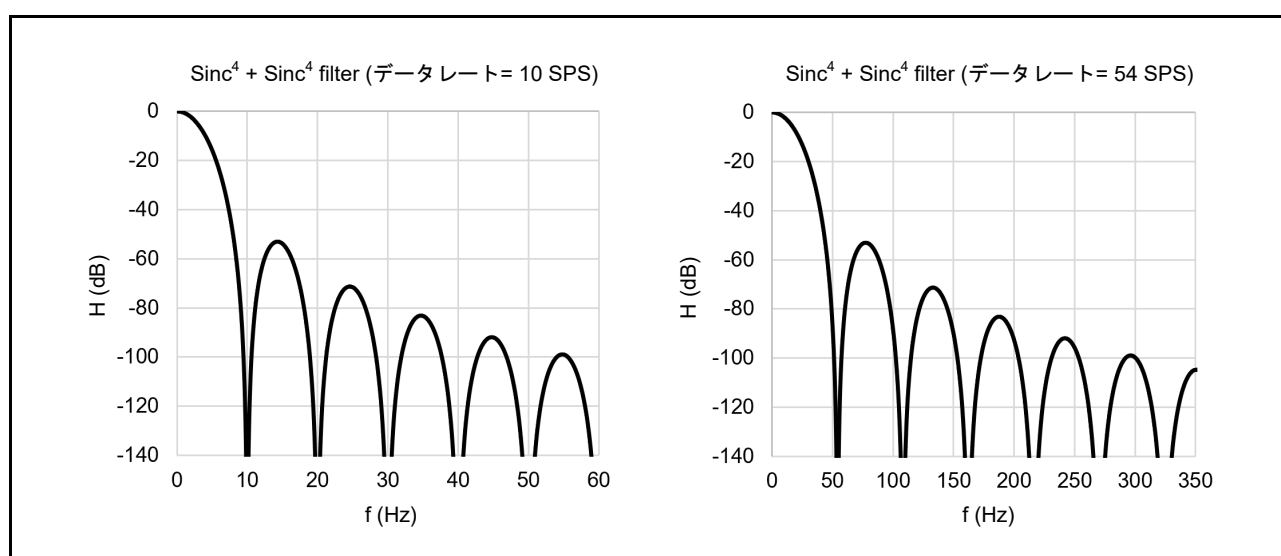
図 36.12 \text{Sinc}^4 + \text{Sinc}^4 フィルタ周波数応答
