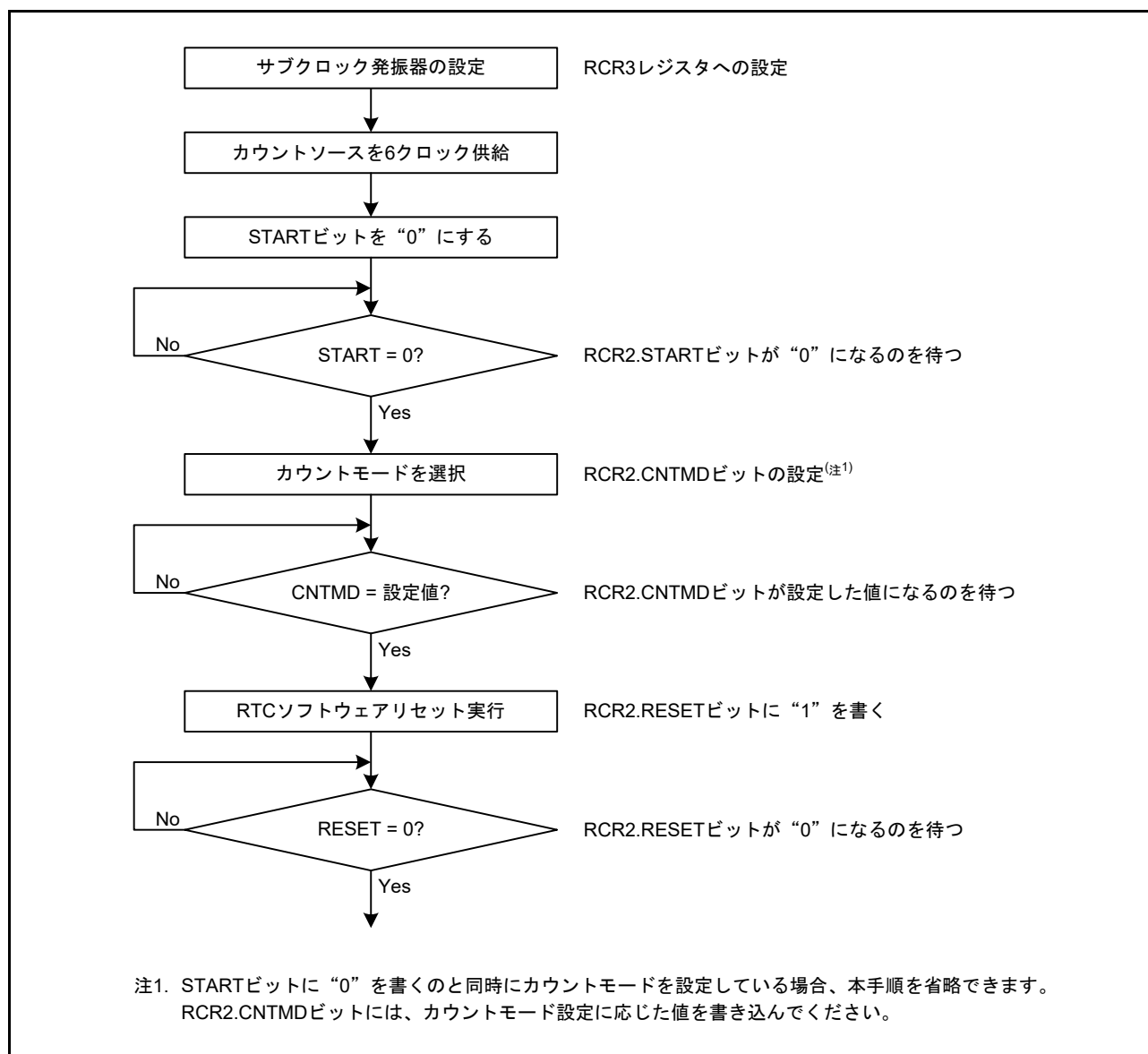
図 26.3 クロック設定手順
