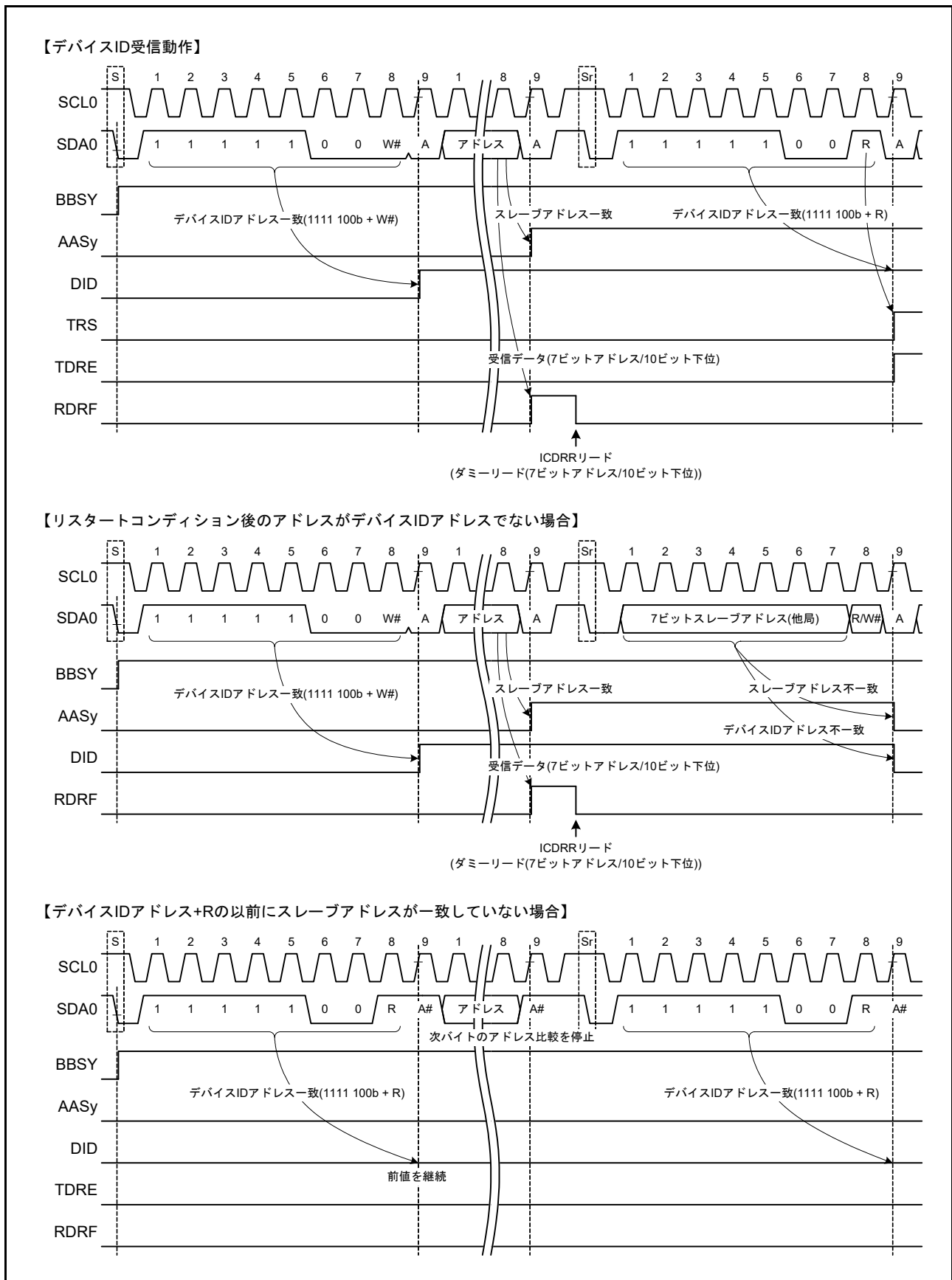
図 30.27 デバイス ID アドレス受信時の AASy、DID フラグセット / クリアタイミング
