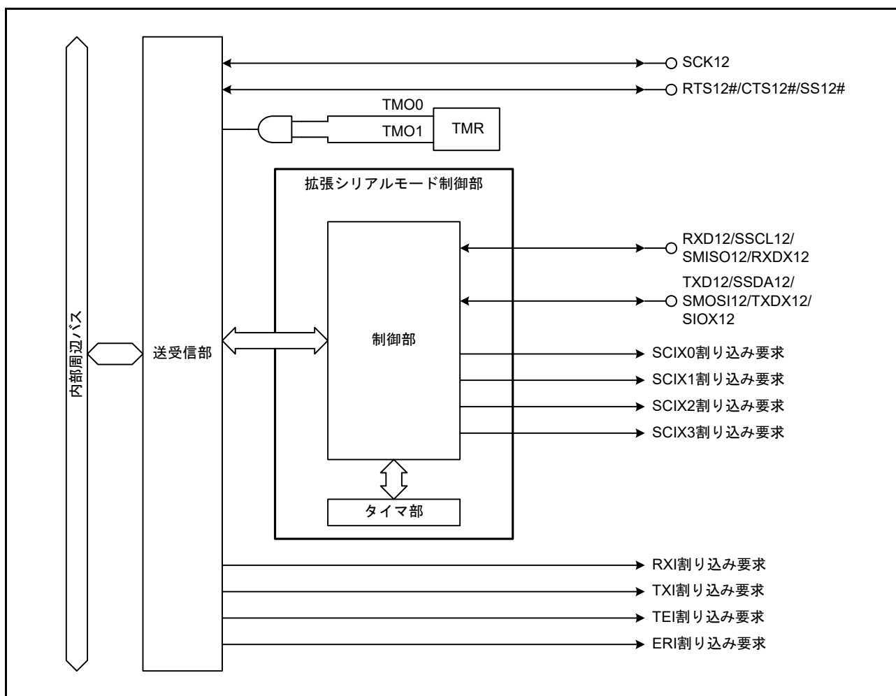
図 29.3 SCIf (SCI12) のブロック図
