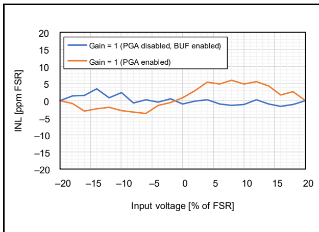
図 42.80 積分非直線性誤差の入力電圧依存性 ( AVCC0 = 5.0V 、 T_a = 25^\circ C 、 f_{MOD} = 4MHz 、 総合 OSR = 4096 、 V_{REF} = 2.5V )
