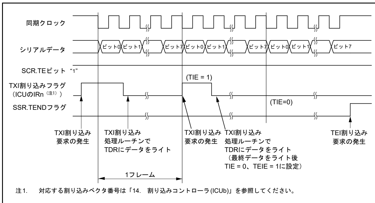
図 29.27 クロック同期式モードのシリアル送信の動作例 (3) (送信中～送信終了時)
