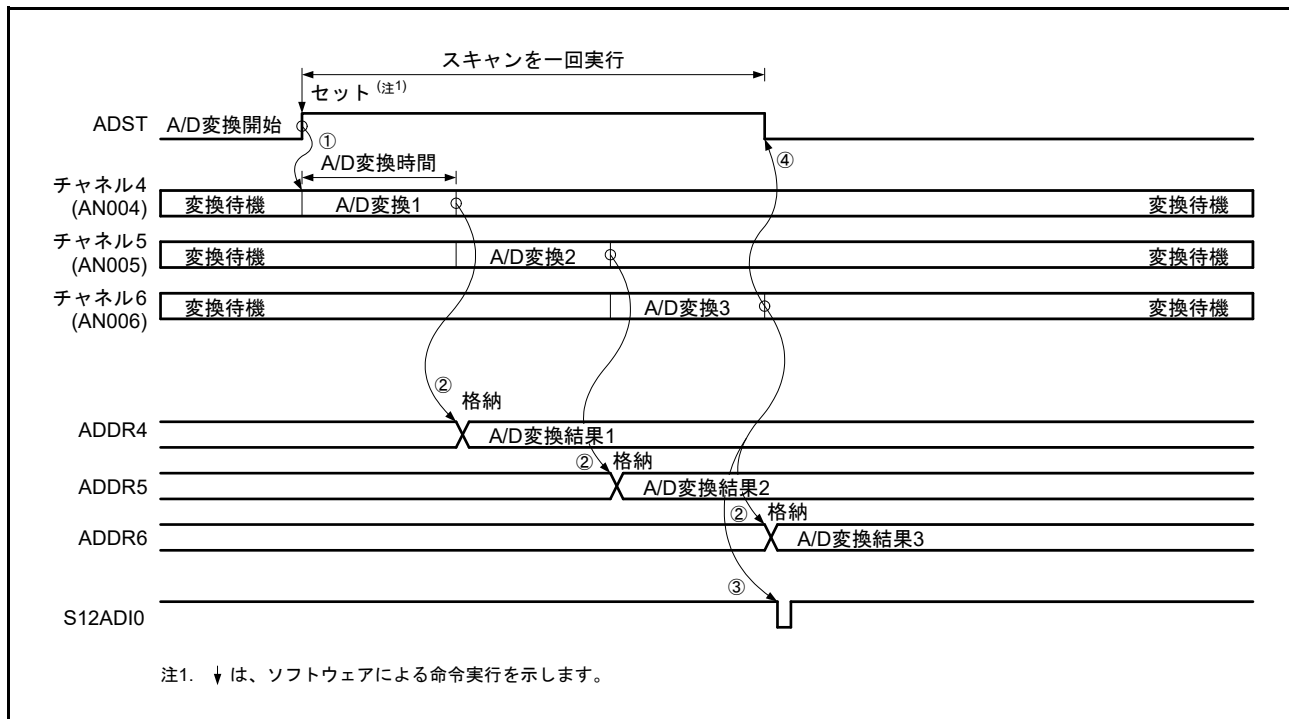
図 37.5 シングルスキャンモードの動作例 (基本動作 : AN004、AN005、AN006 選択)
