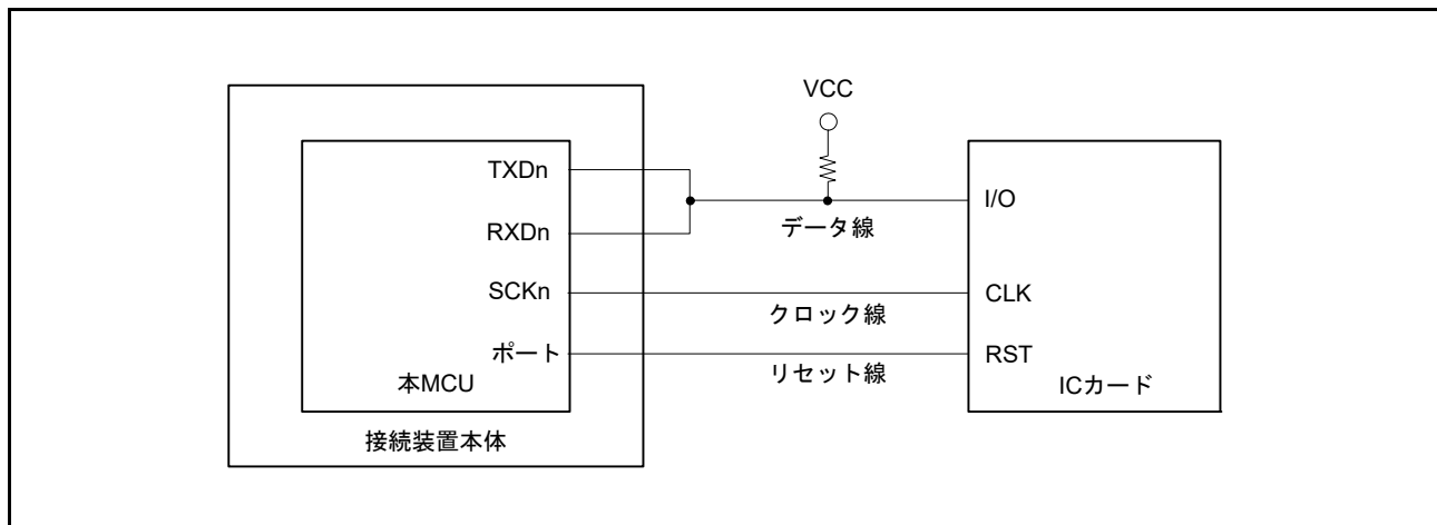
図 29.33 スマートカード (IC カード) との接続例
