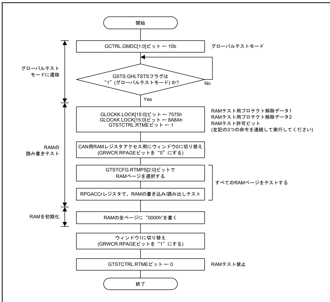
図 31.35 RAMテストの設定手順
