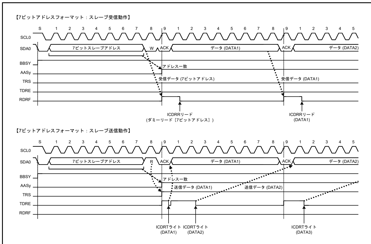
図 30.23 7ビットアドレスフォーマット選択時にAASyフラグが“1”になるタイミング
