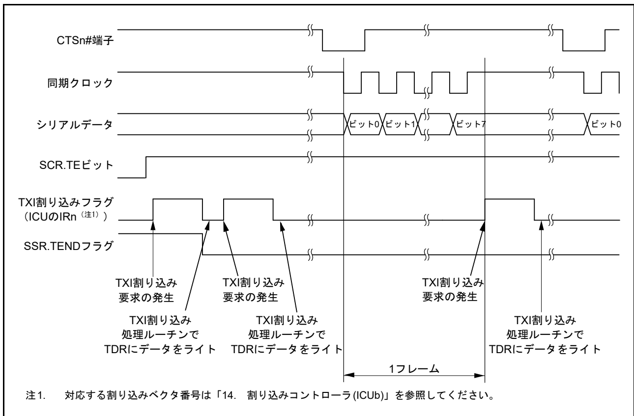
図 29.26 クロック同期式モードのシリアル送信の動作例 (2) (送信開始・CTS 機能使用する)
