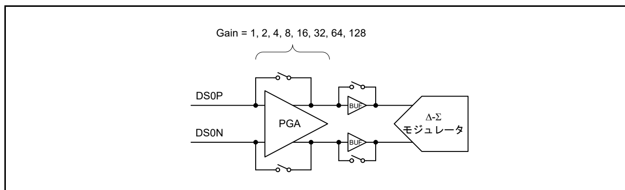
図 36.3 プログラマブルゲイン計装アンプの接続
