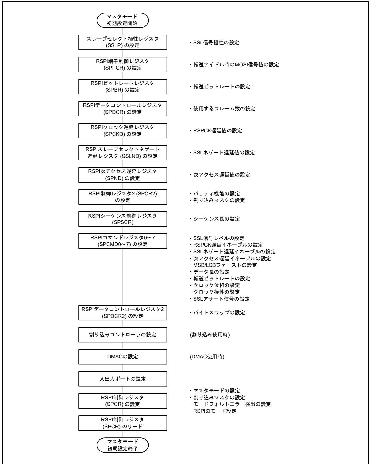
図 32.37 マスターモード時の初期化フロー例 (SPI 動作)
