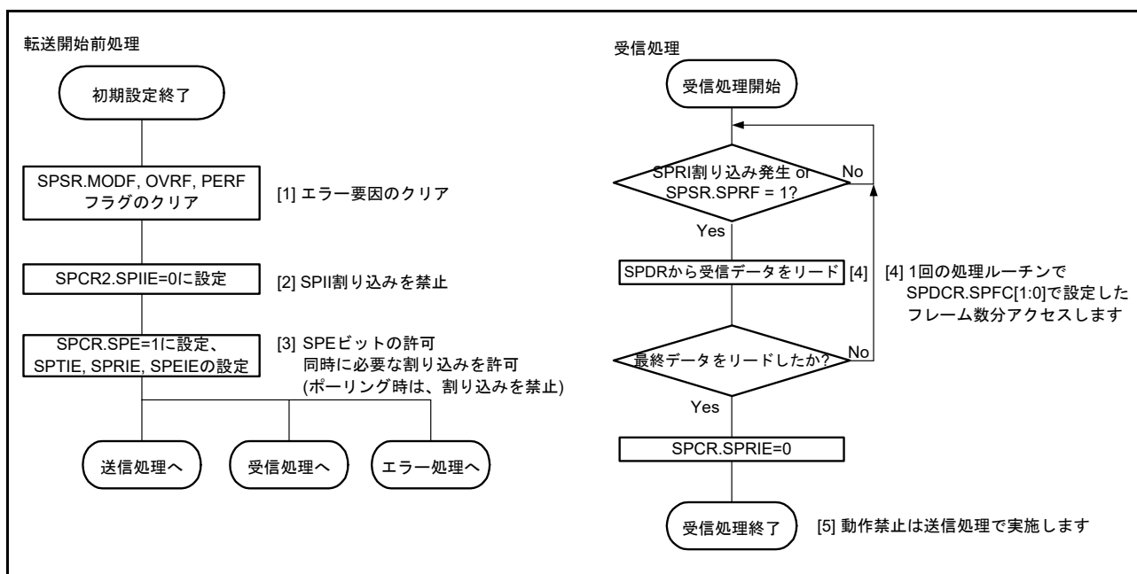
図 32.39 マスタモード時のフローチャート (受信)
