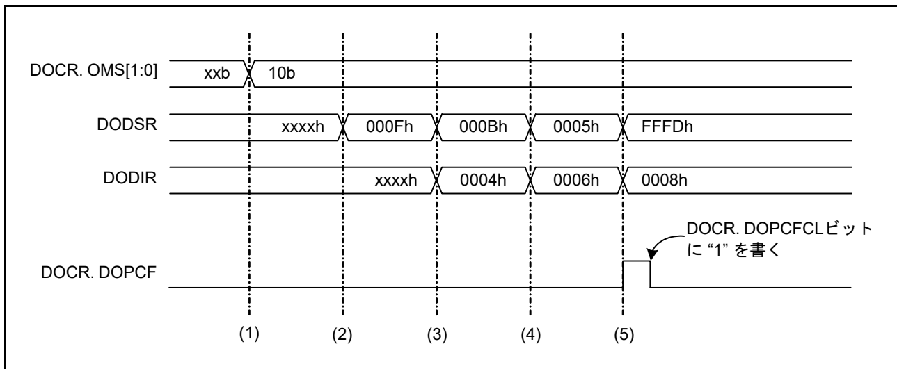
図 39.4 データ減算モードの動作例
