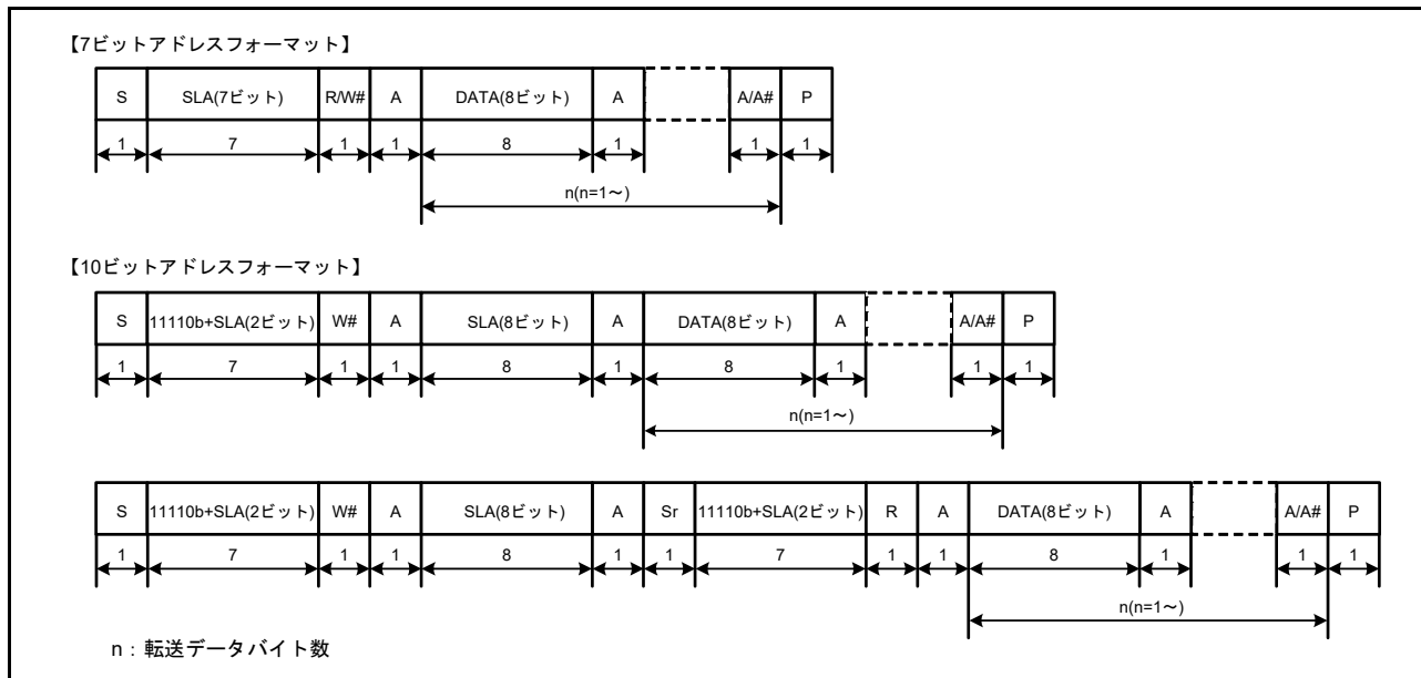
図 30.2 I 2 C バスフォーマット
