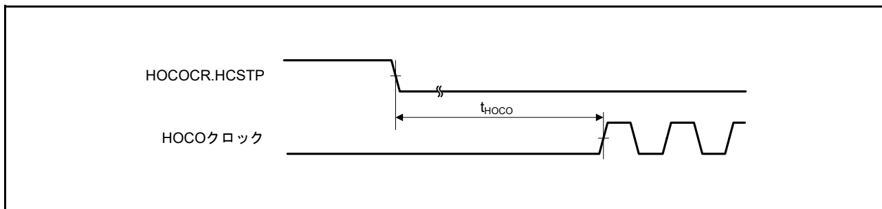
図 42.21 HOCO クロック発振開始タイミング (HOCOCR.HCSTP ビット設定による発振開始)
