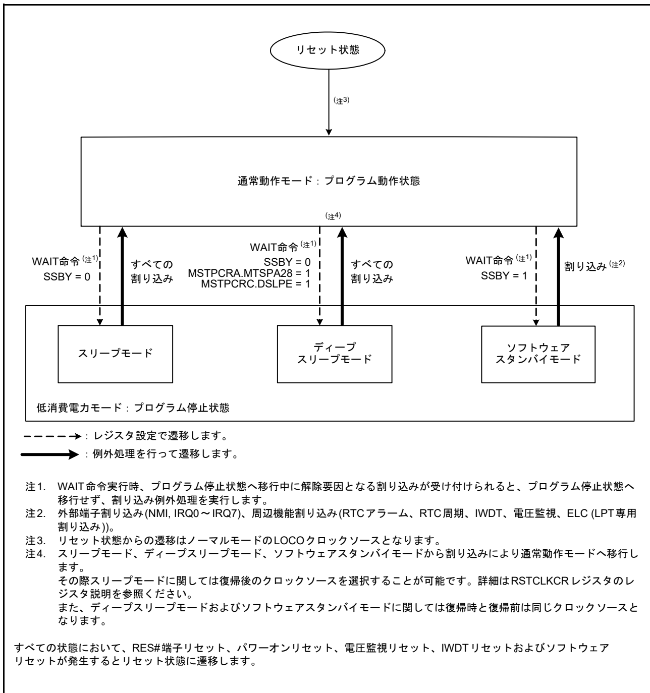
図 11.1 モード遷移
