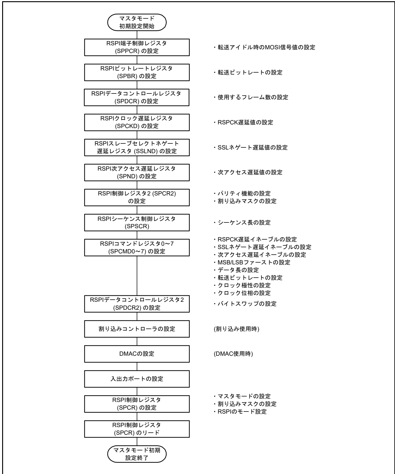
図 32.48 マスターモード時の初期化フロー例 (クロック同期式動作)
