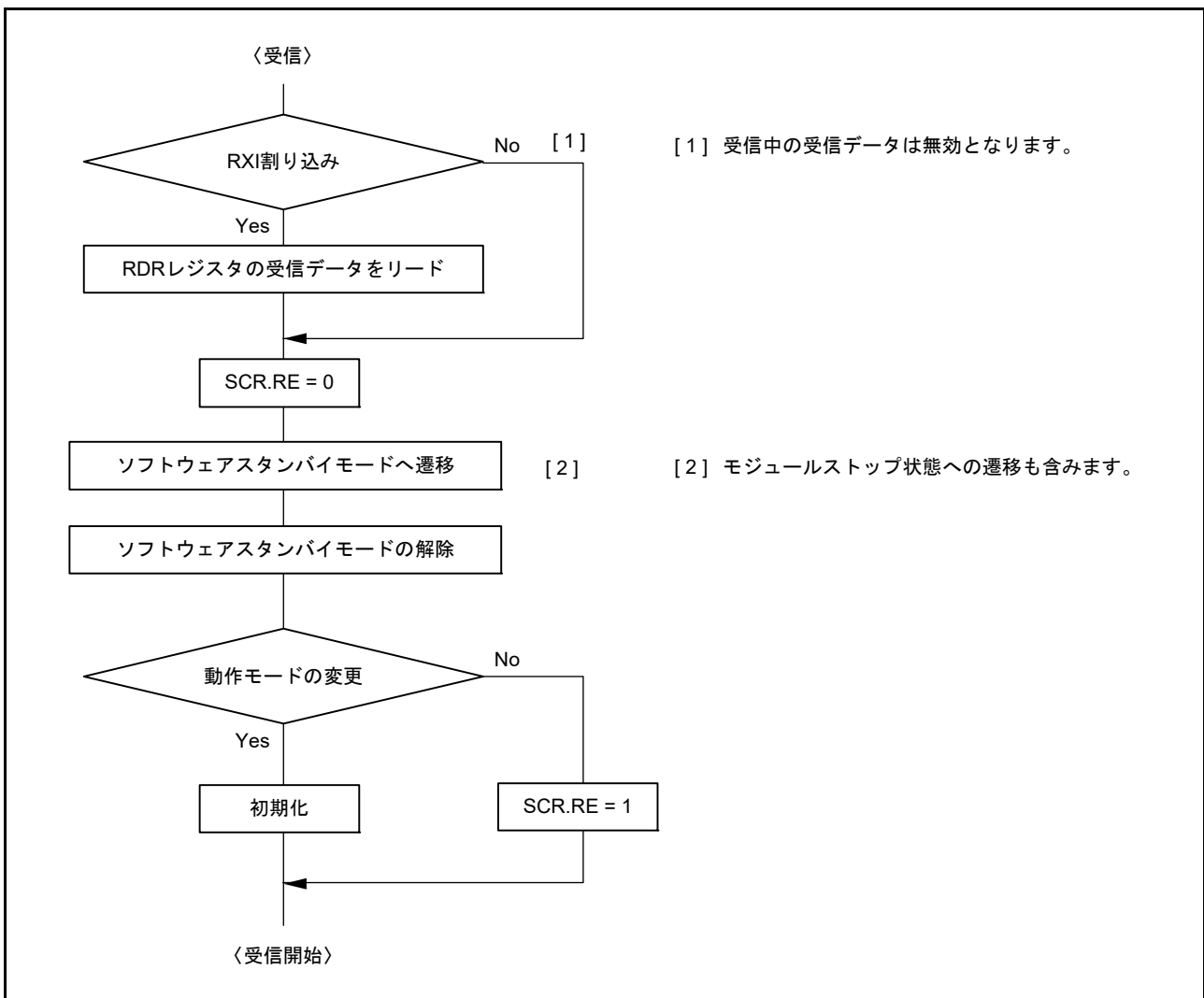
図 29.80 受信時のソフトウェアスタンバイモード遷移フローチャートの例
