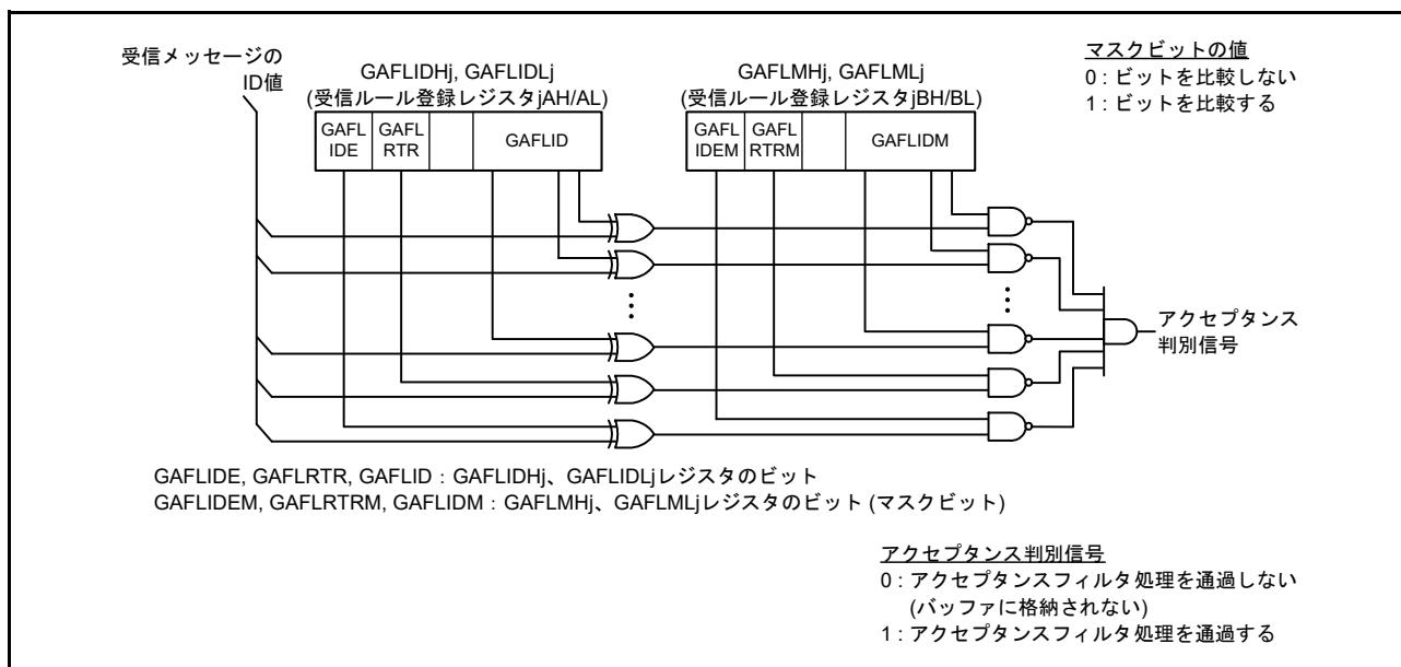
図 31.5 アクセプタンスフィルタ機能
