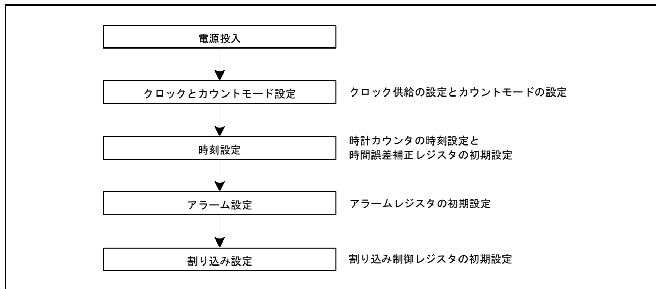
図 26.2 電源投入後の初期設定概要
