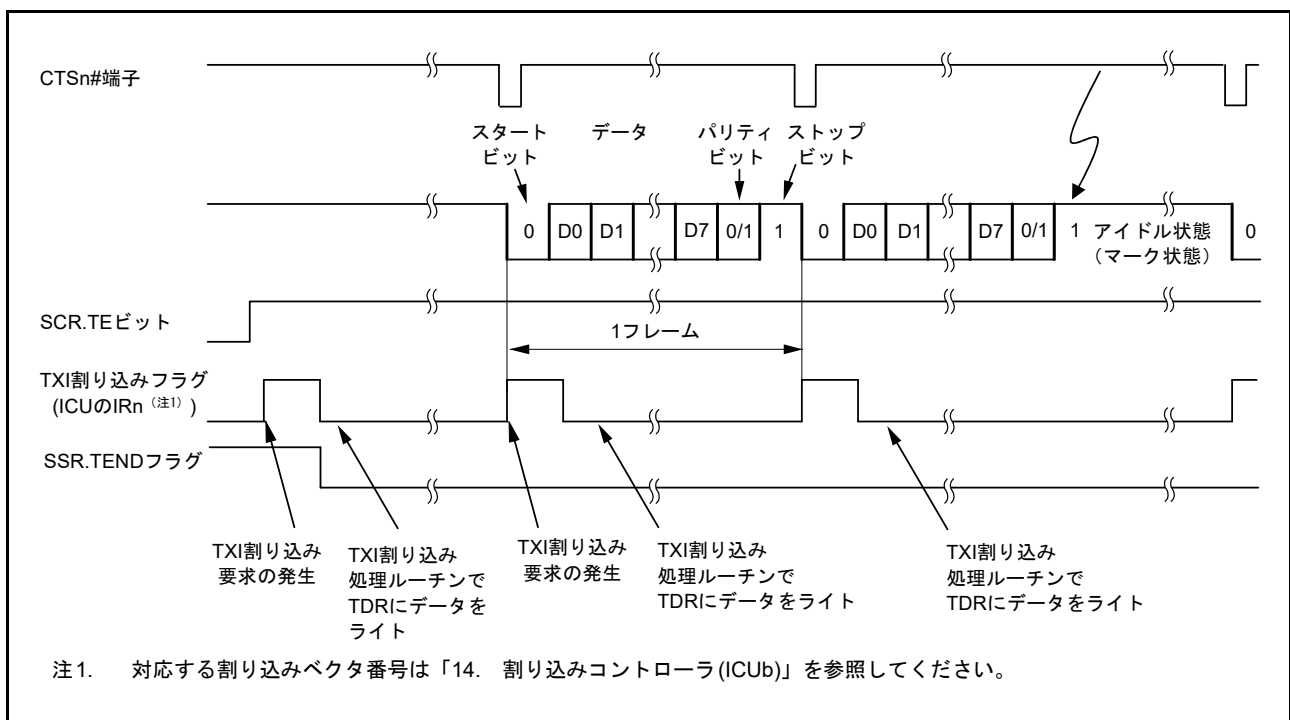
図 29.11 調歩同期式モードのシリアル送信の動作例 (2) (8ビットデータ / パリティあり / 1ストップビット / CTS 機能使用する / 送信開始時)
