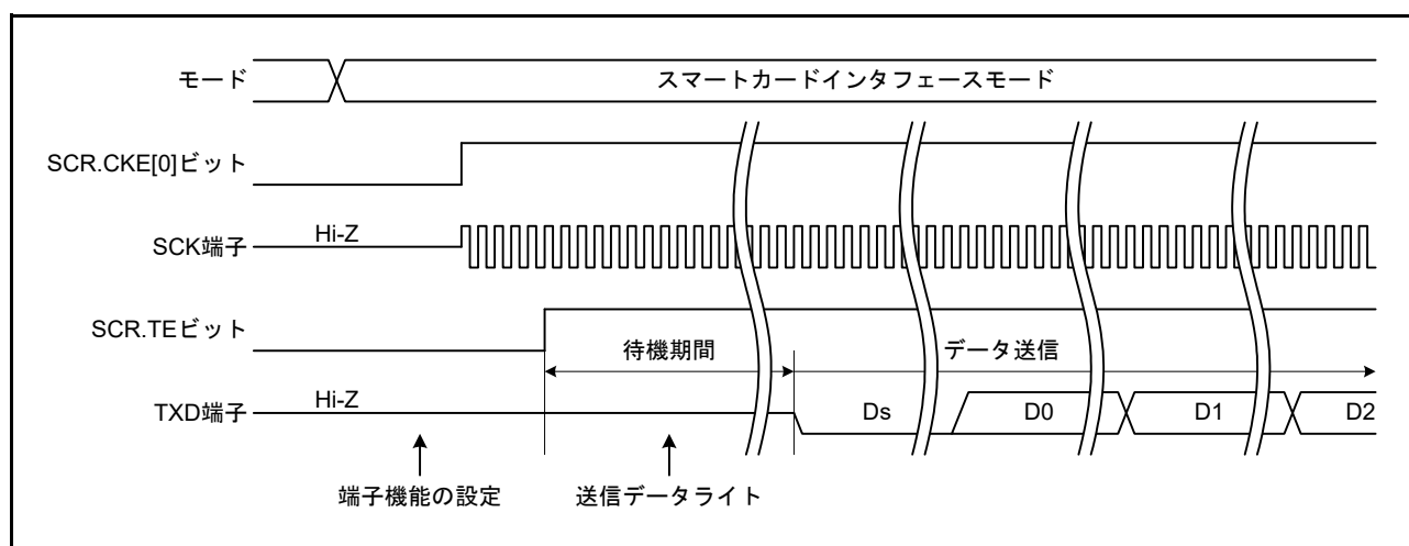
図 29.39 スマートカードインタフェースモード時のデータ送信タイミング例
