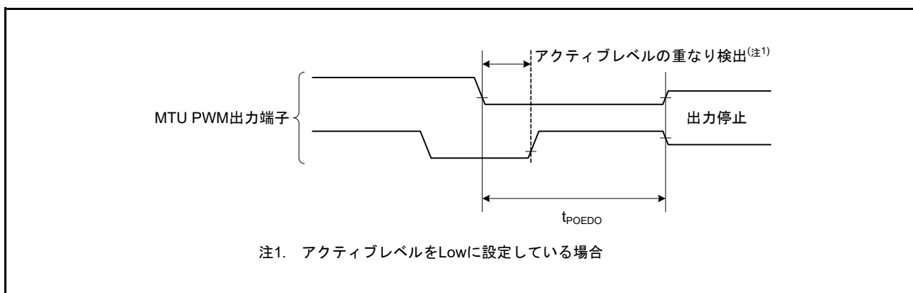
図 42.36 POE 出力ディセーブル時間 (出力端子の短絡)
