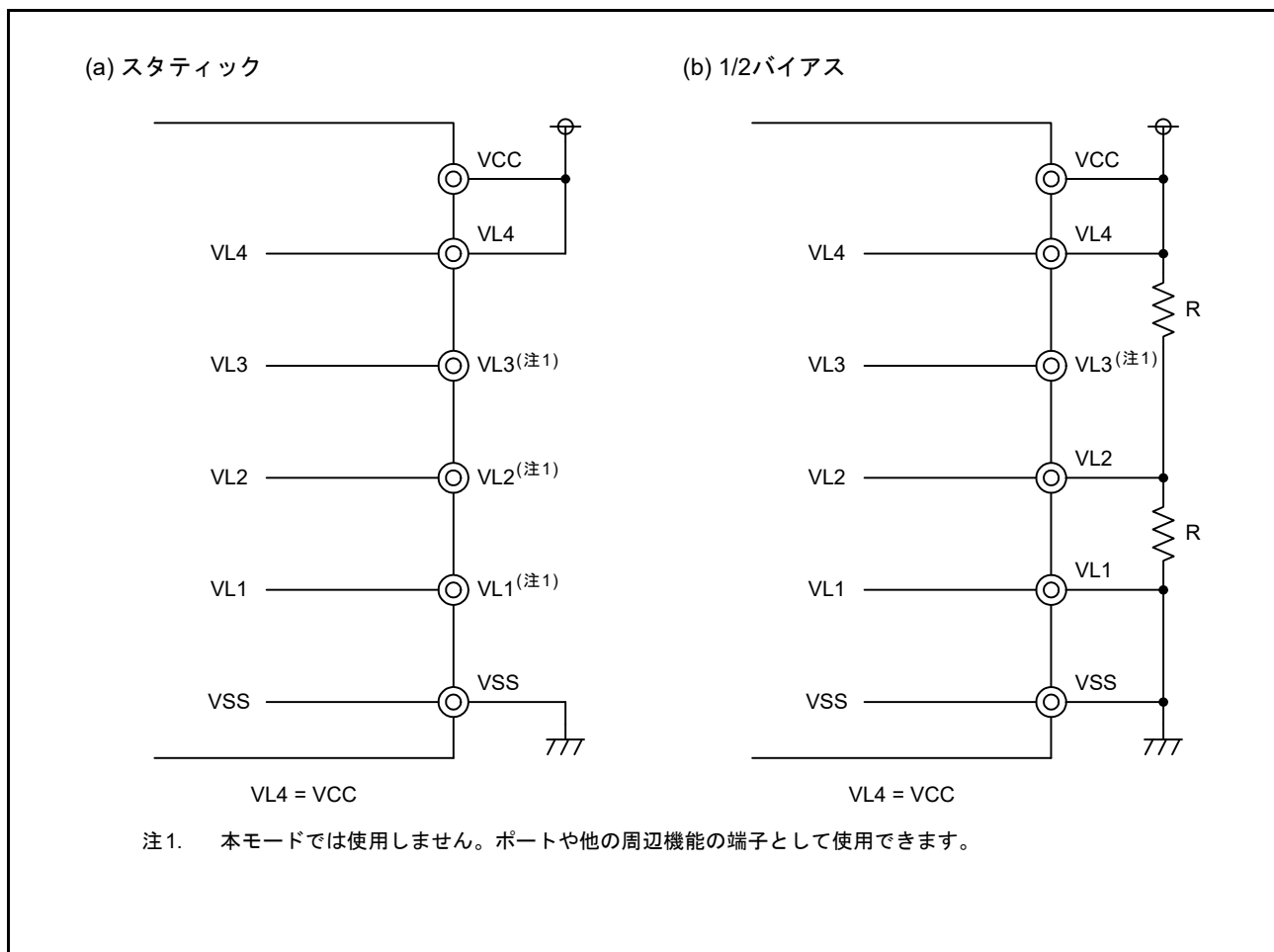
図 34.9 LCD バイアス電圧の供給例 (外部抵抗分割方式) (1)
