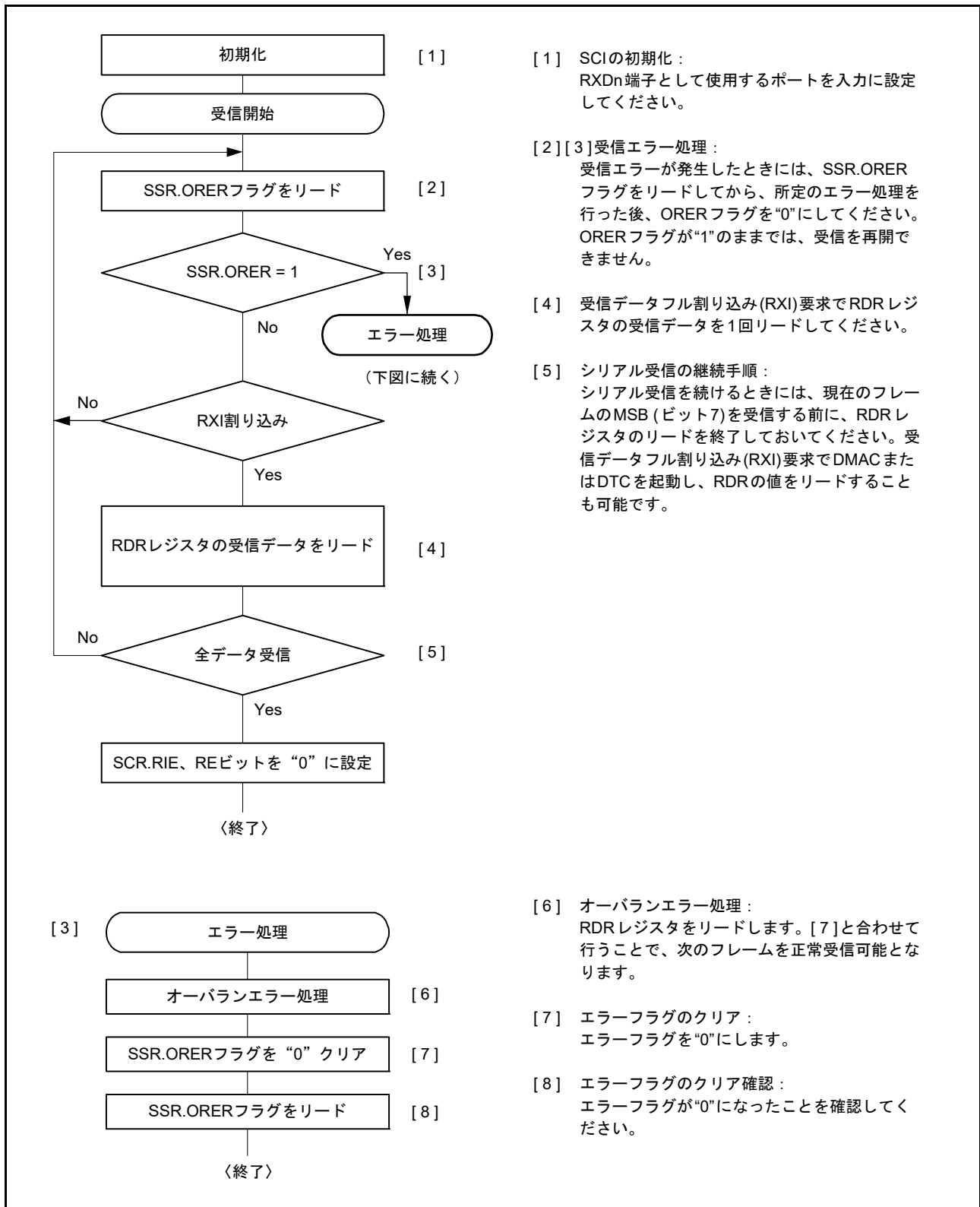
図 29.31 クロック同期式モードのシリアル受信のフローチャート例
