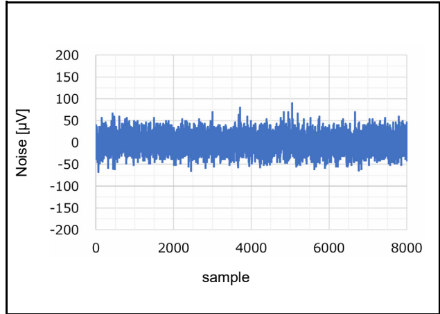
図 42.75 ノイズプロット (AVCC0 = 5.0V、 T_a = 25^\circ\text{C} 、Gain = 1 (PGA 無効、BUF 有効)、 f_{\text{MOD}} = 4\text{MHz} 、 f_{\text{DR}} = 976.6\text{ SPS} 、Sinc 4 +Sinc 4 フィルタ、 V_{\text{ID}} = 0\text{V} 、 V_{\text{REF}} = 2.5\text{V} )
