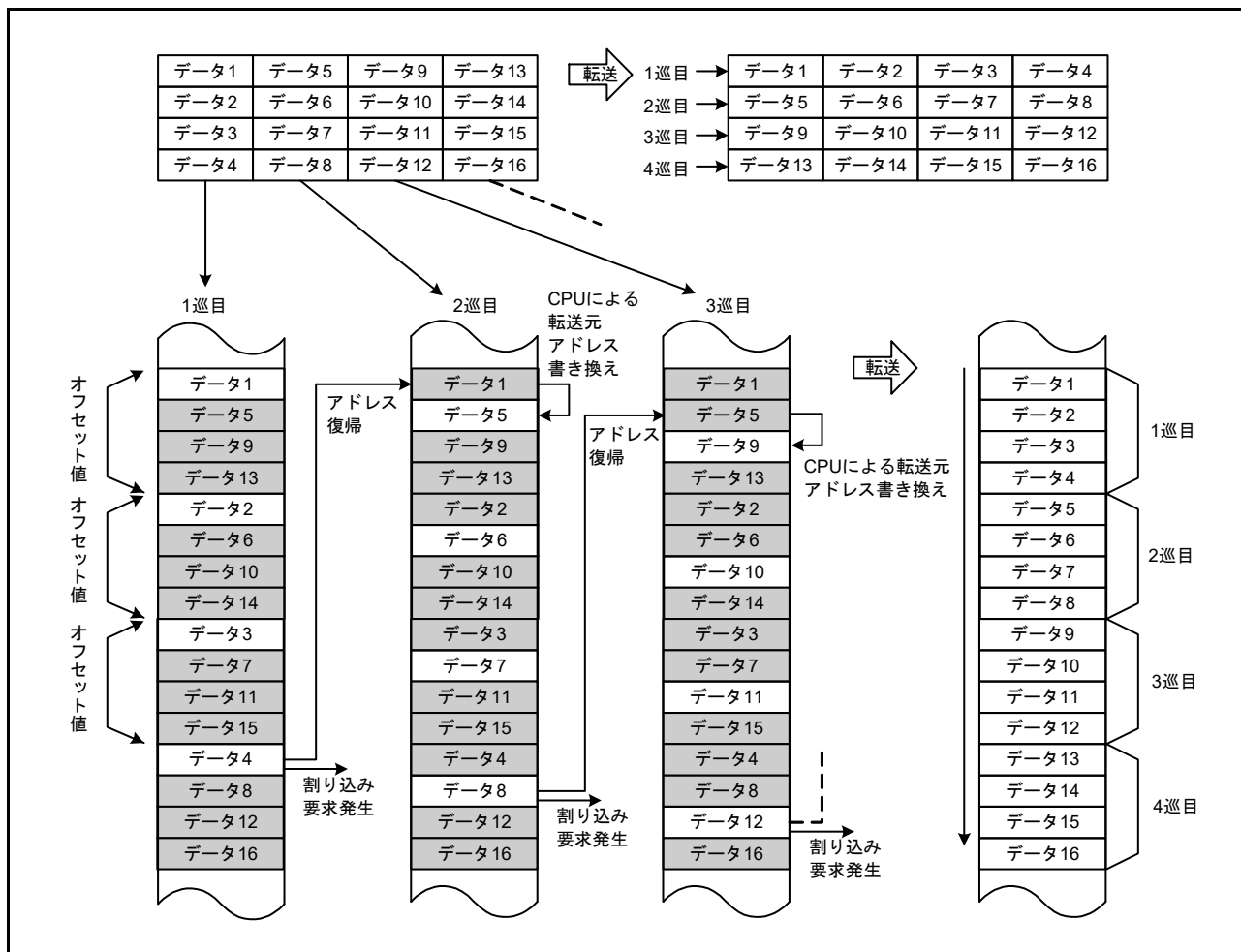
図 17.8 リポート転送モード+オフセット加算によるXY変換のときの動作
