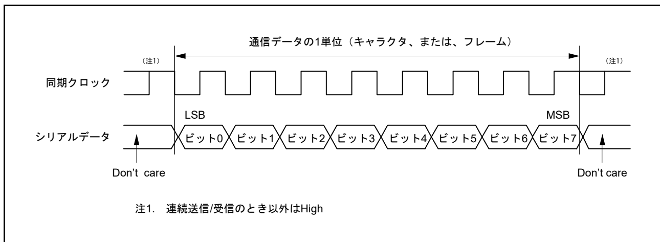
図 29.23 クロック同期式シリアル通信のデータフォーマット (LSB ファーストの場合)
