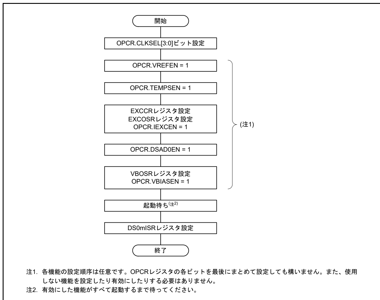
図 35.15 AFEの初期化フロー
