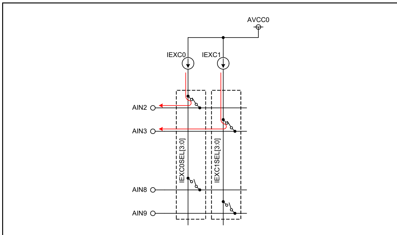
図 35.9 IEXC の設定例
