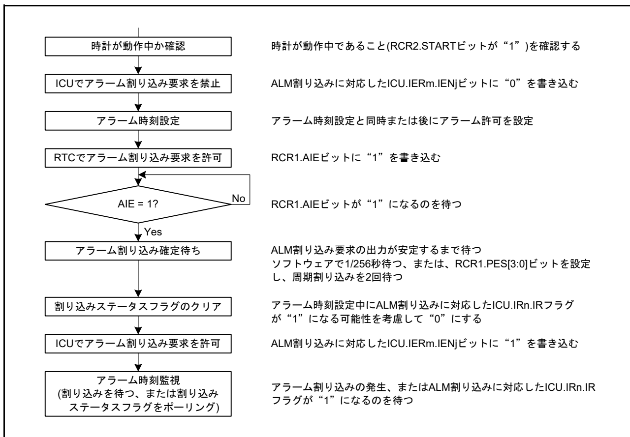
図 26.7 アラーム機能の使用方法
