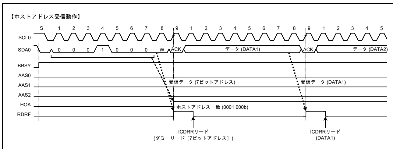
図 30.28 ホストアドレス受信時に HOA フラグが“1”になるタイミング
