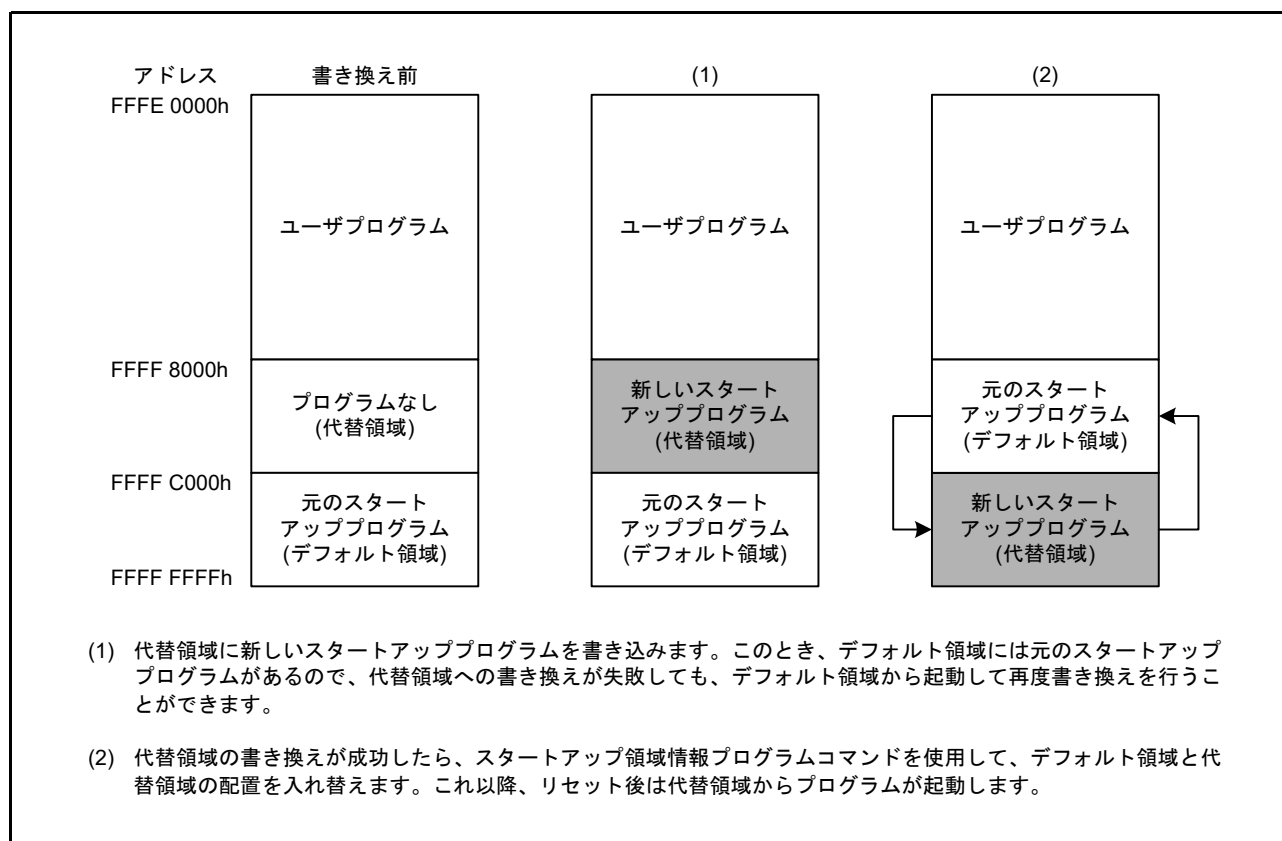
図 41.4 スタートアッププログラム保護機能の概念
