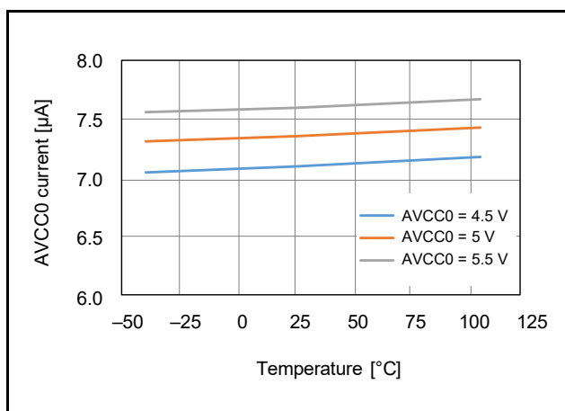
図 42.7 24 ビット \Delta - \Sigma A/D コンバータ動作電流の温度依存性 (PGA 無効、BUF 無効)
