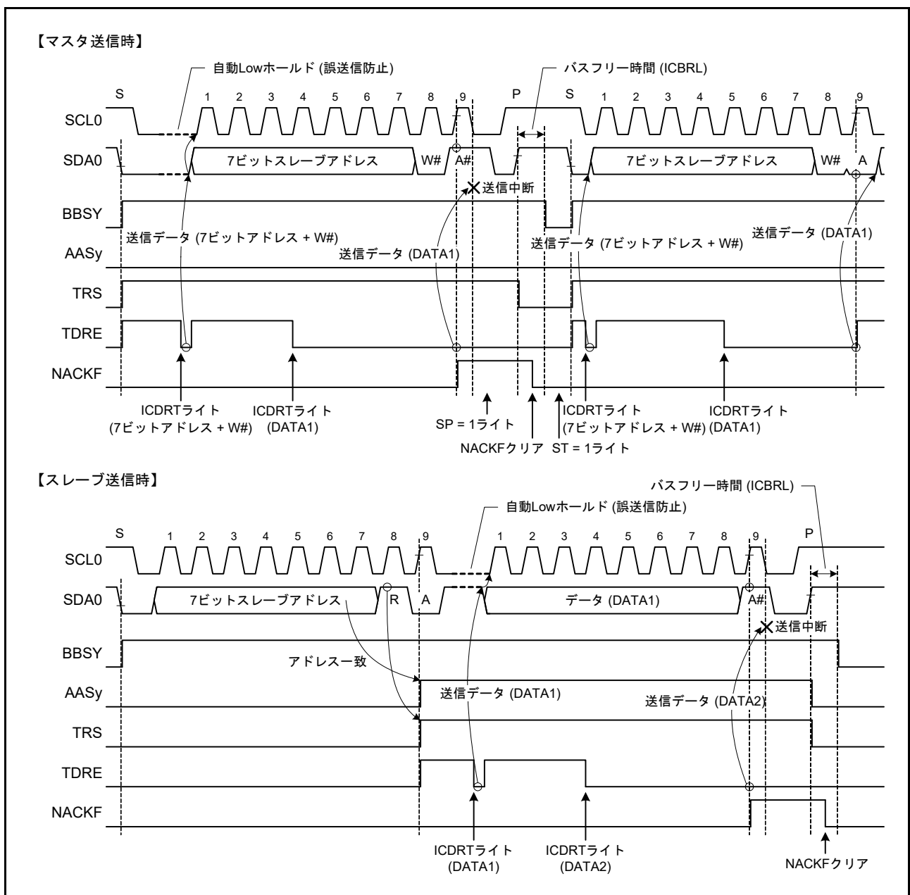
図 30.30 NACK 受信時の転送中断動作 (NACKE ビット = 1 のとき)
