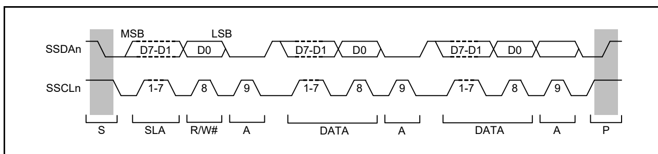
図 29.47 I 2 C バスタイミング (SLA = 7 ビットの場合)
