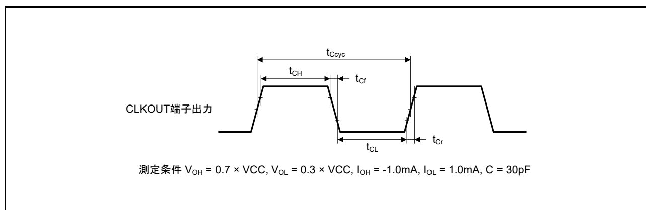
図 42.49 CLKOUT 出力タイミング
