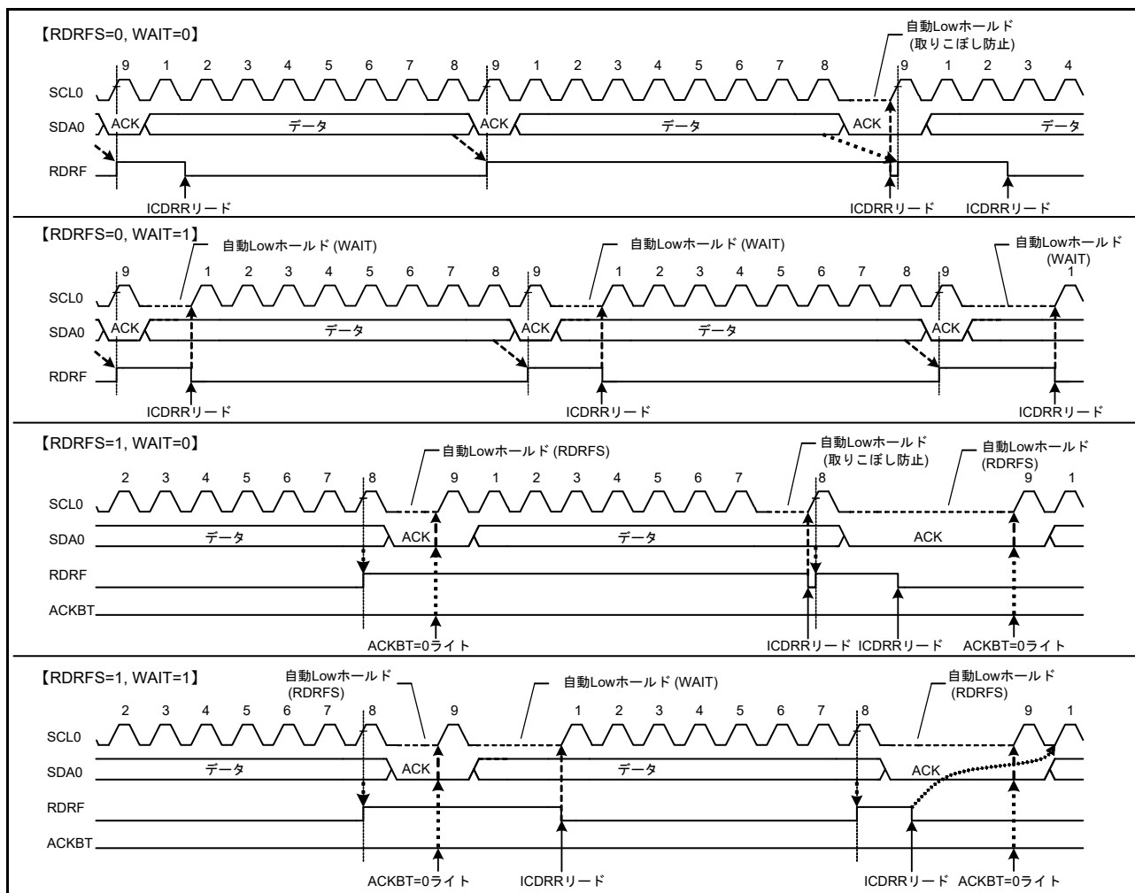
図 30.31 受信モードの自動 Low ホールド動作 (RDRFS、WAIT ビット)
