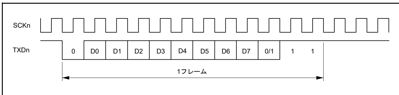
図 29.7 出カクロックと送信データの位相関係 (調歩同期式モード: SMR.CHR = 0、PE = 1、MP = 0、STOP = 1)
