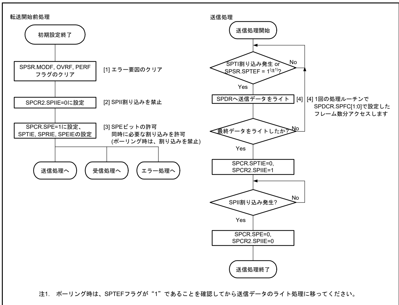
図 32.38 マスタモード時のフローチャート (送信)
