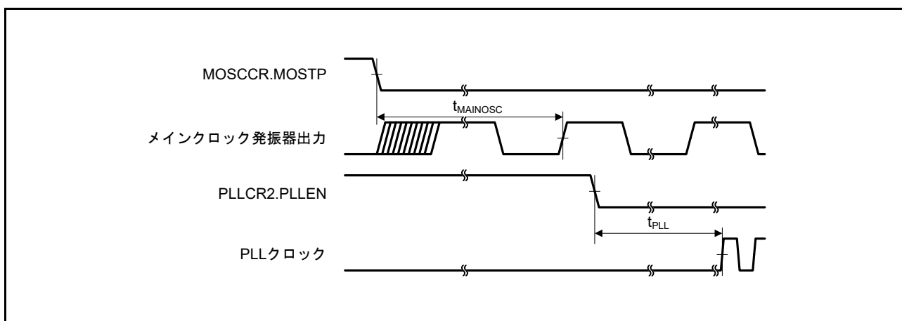
図 42.22 PLL クロック発振開始タイミング (メインクロック発振安定後に PLL を動作させたとき)
