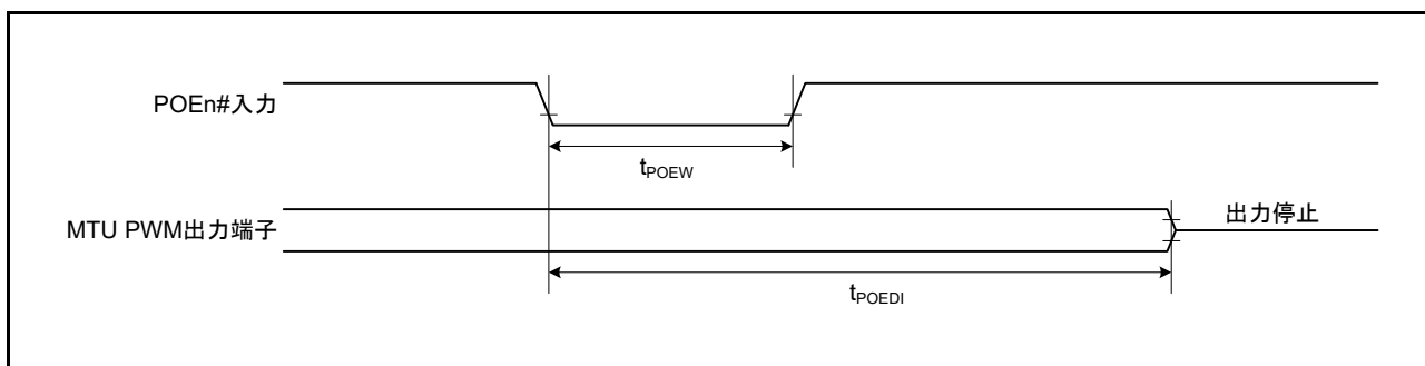
図 42.35 POE 出力ディセーブル時間 (POEn# 端子の変化)
