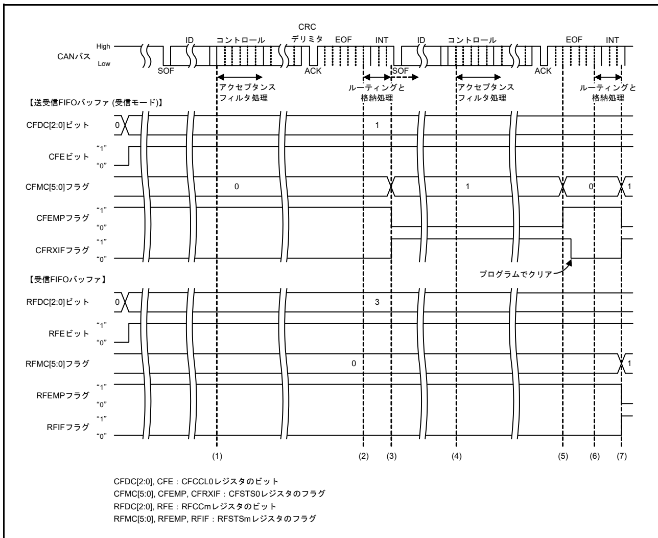
図 31.25 FIFO バッファの受信タイミング図
