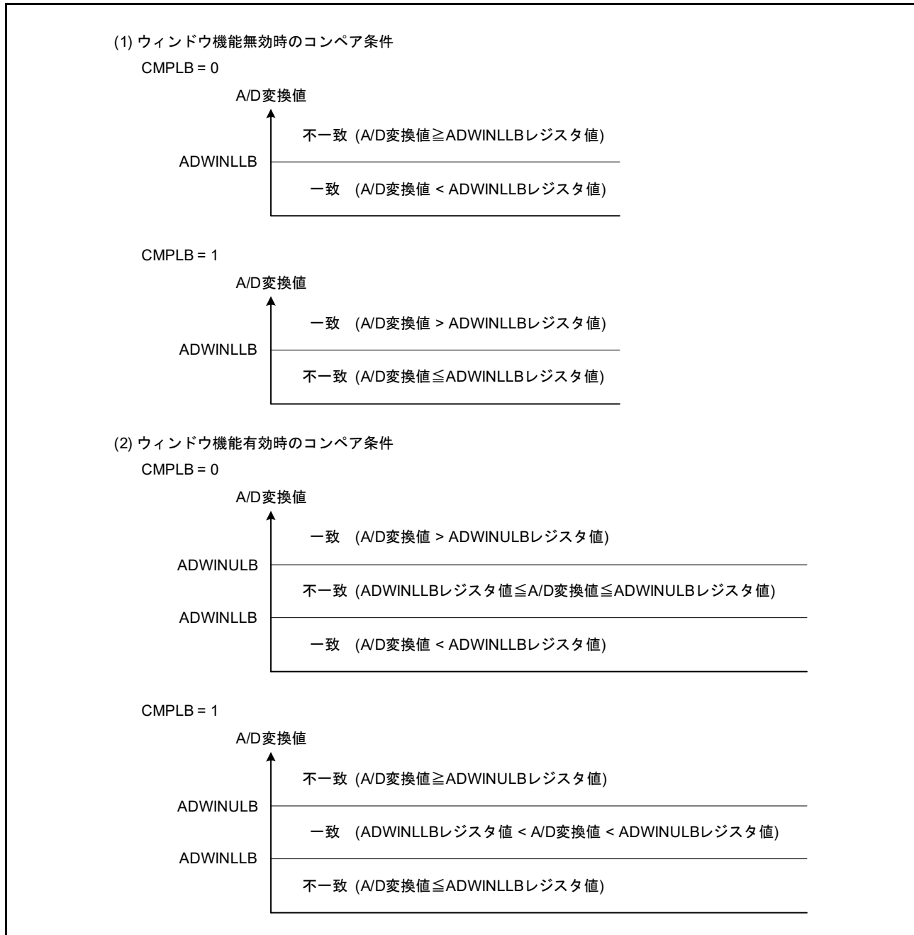
図 37.4 コンペア機能ウィンドウ B コンペア条件説明
