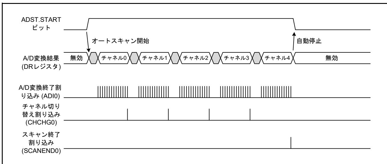
図 36.10 シングルスキャン動作
