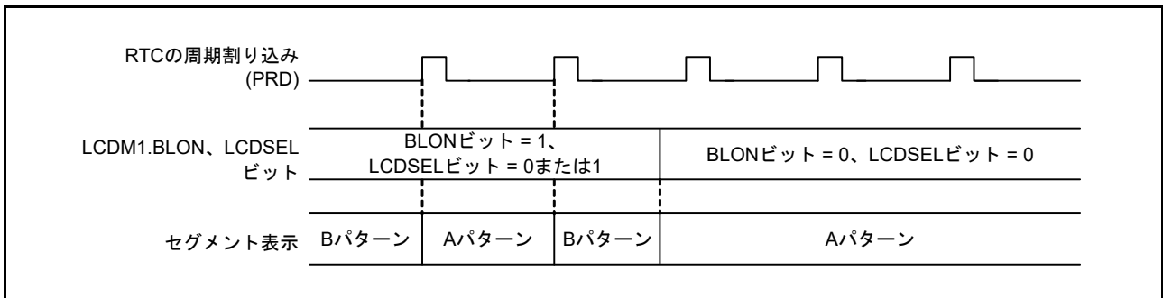
図 34.4 A-B 交互表示から Aパターン領域表示への切り替え動作
