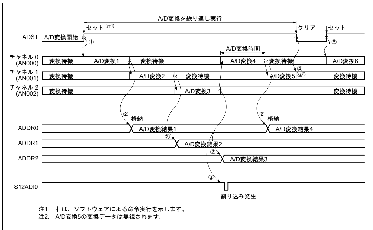
図 37.8 連続スキャンモードの動作例 (基本動作 : AN000、AN001、AN002 選択)
