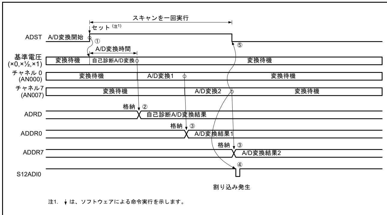
図 37.6 シングルスキャンモードの動作例 (基本動作 : AN000、AN007 選択 + 自己診断)
