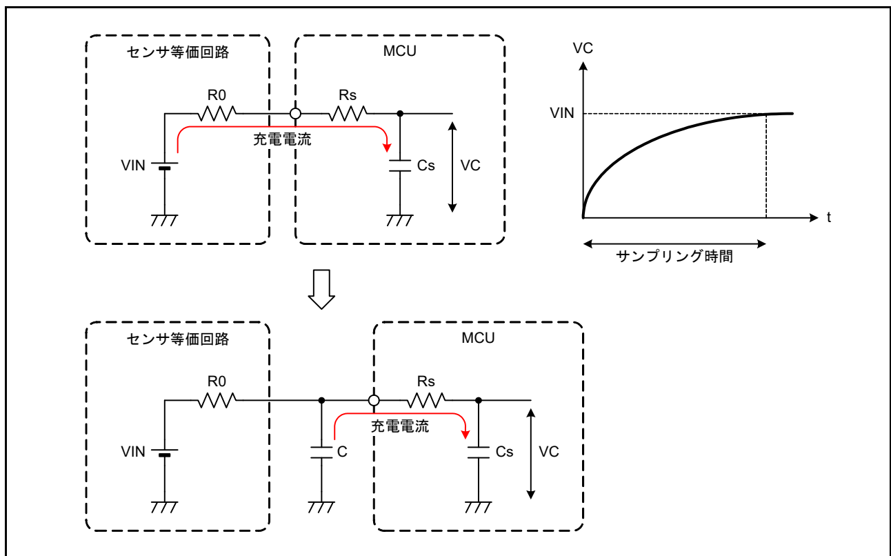
図 37.27 アナログ入力端子と外部センサの等価回路
