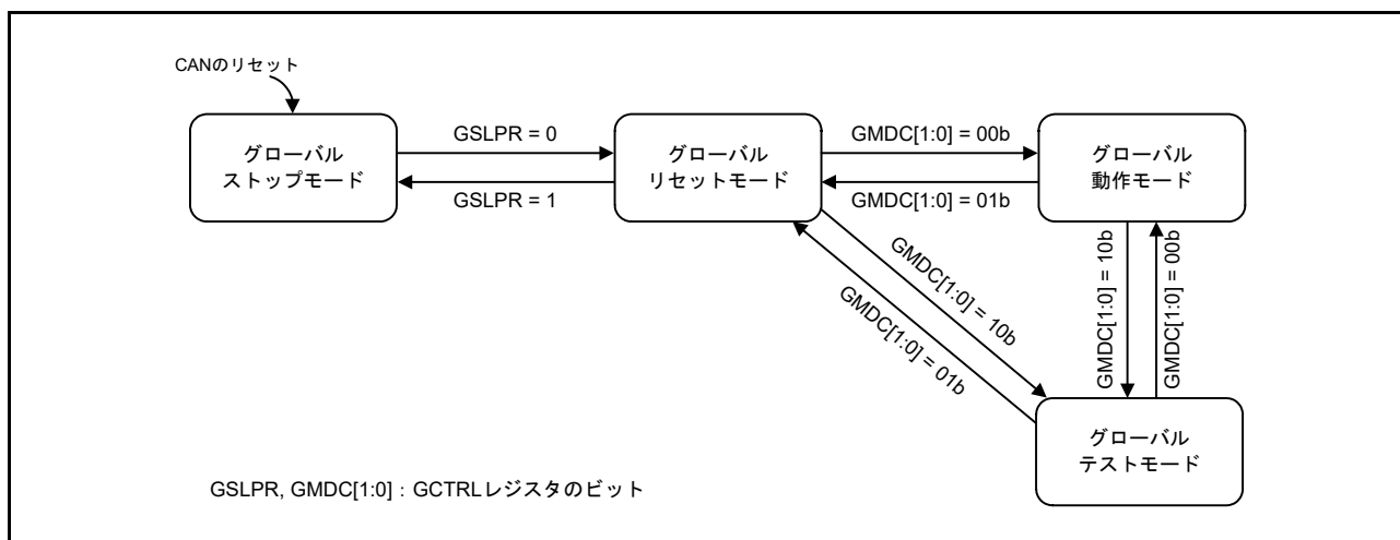
図31.2 グローバルモードの遷移図
