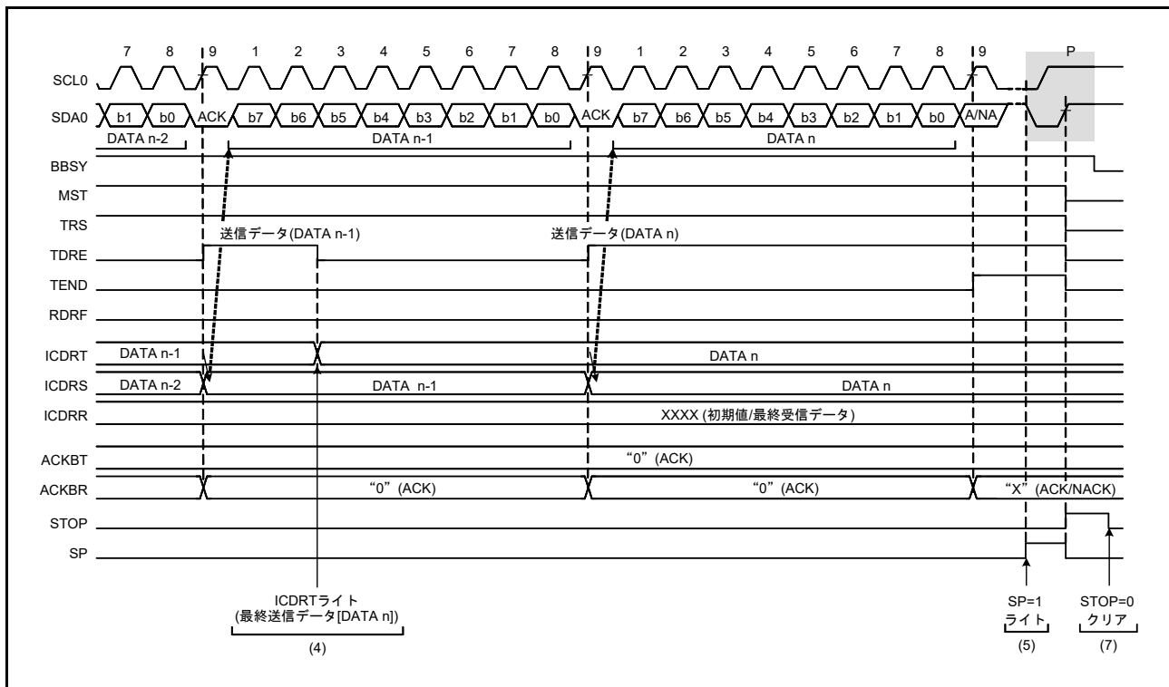
図 30.8 マスタ送信の動作タイミング (3)
