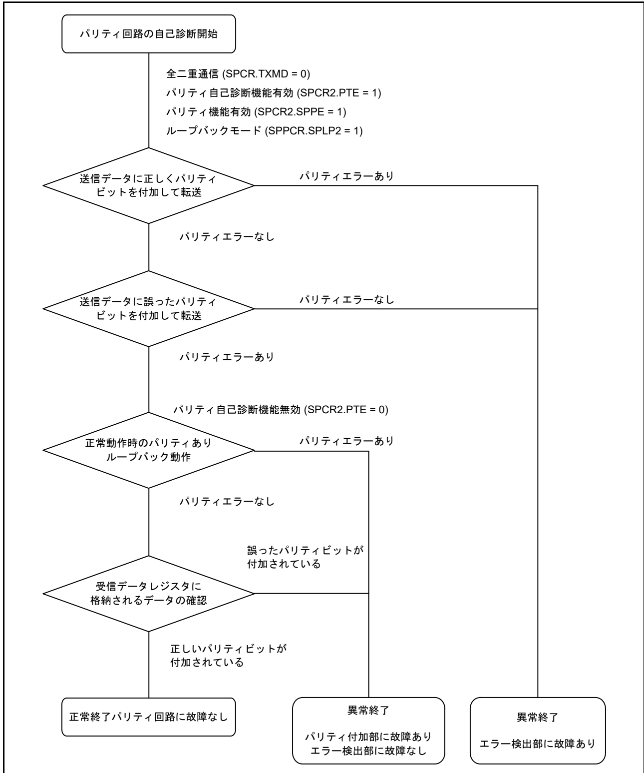
図 32.51 パリティ回路の自己判断フロー
