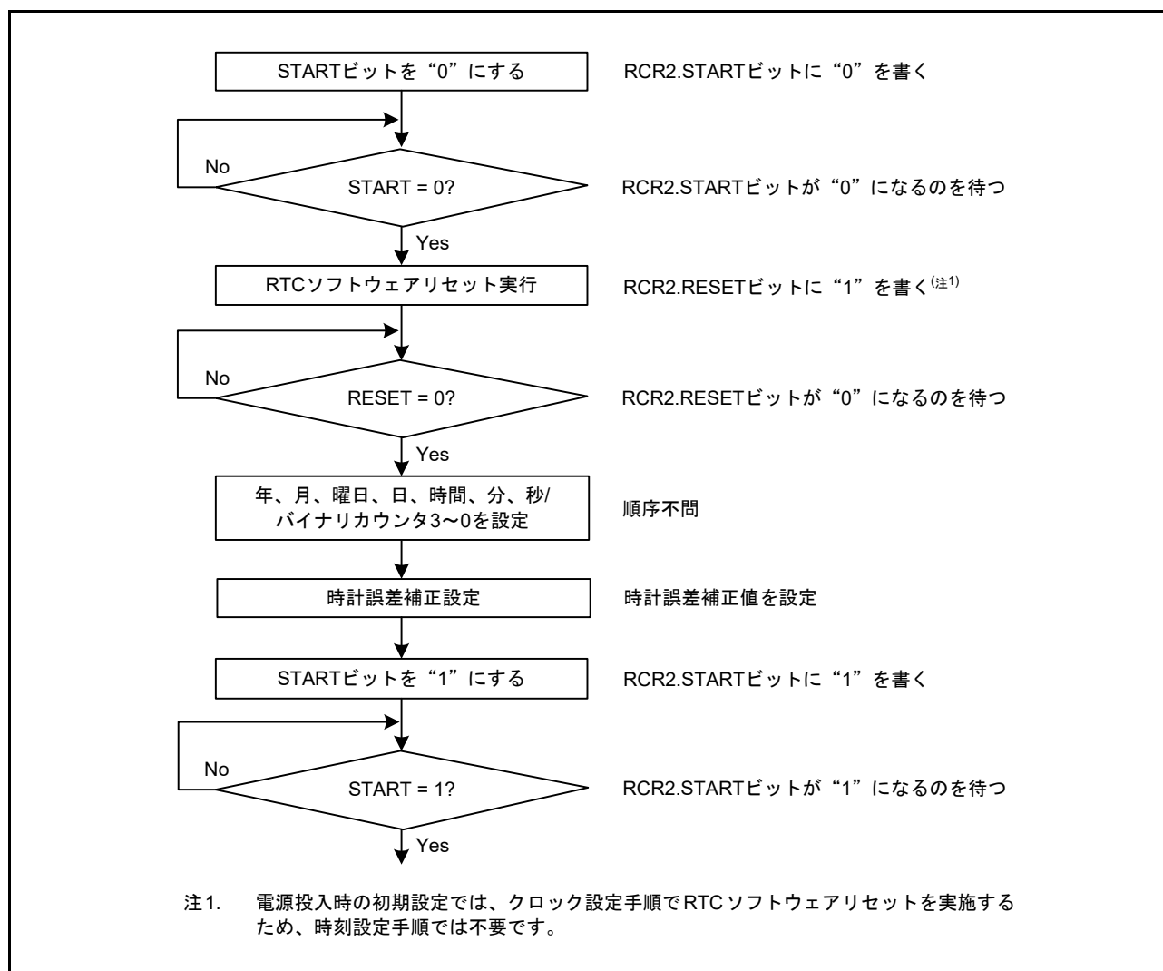
図 26.4 時刻設定手順
