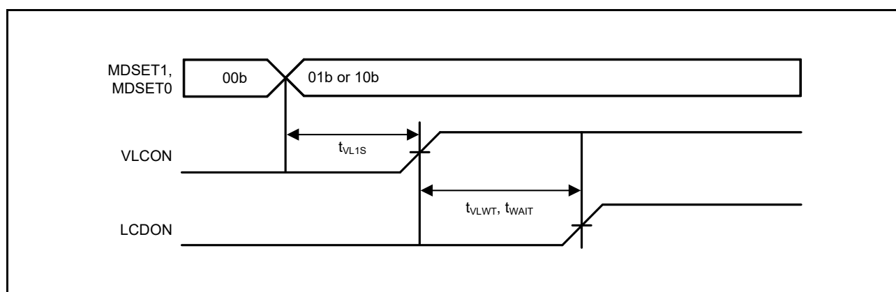
図 42.50 LCD 基準電圧セットアップ時間と昇圧ウェイト時間と容量分割ウェイト時間
