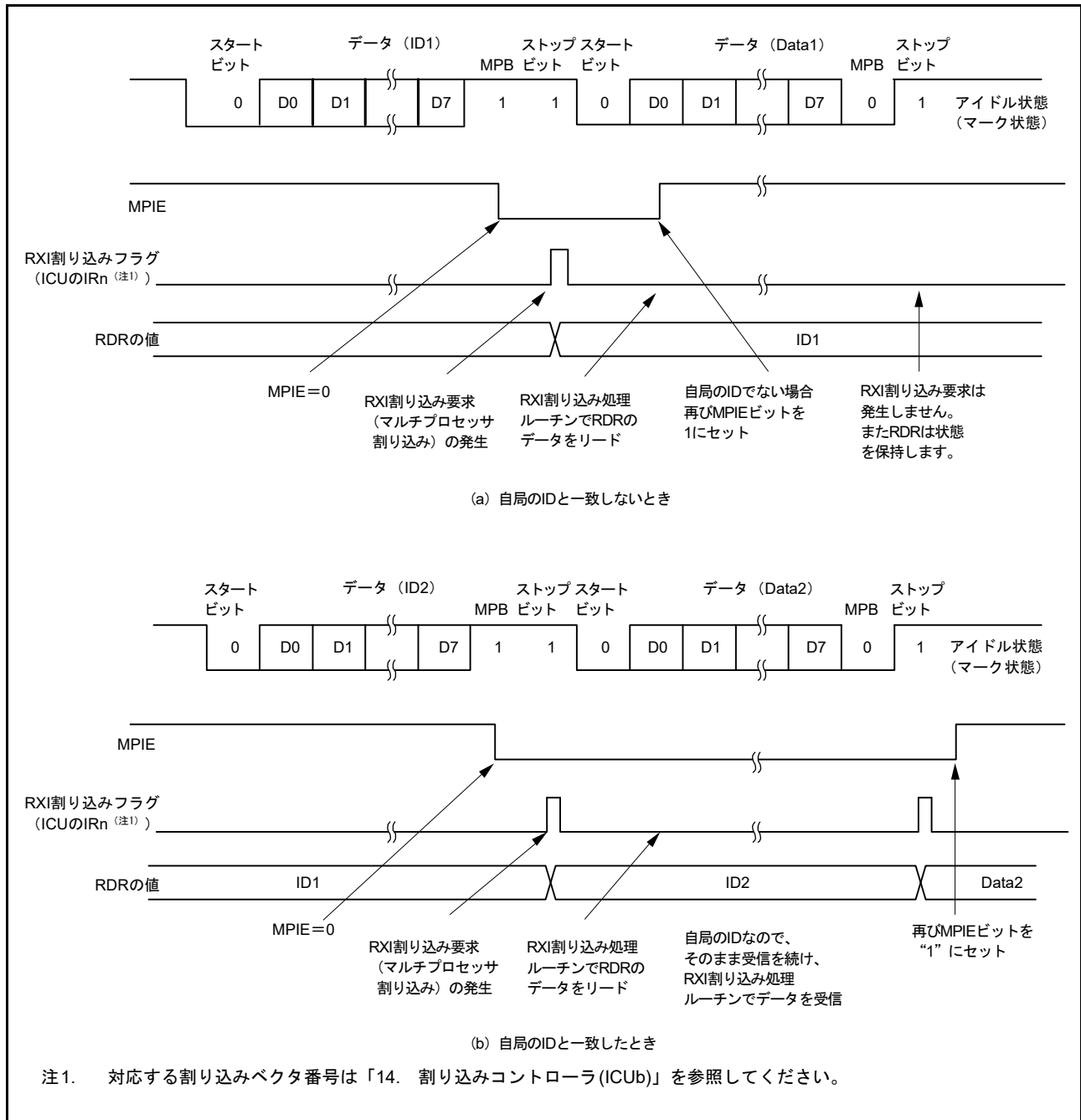
図 29.20 SCI の受信時の動作例 (8 ビットデータ / マルチプロセッサビットあり / 1 ストップビットの例)
