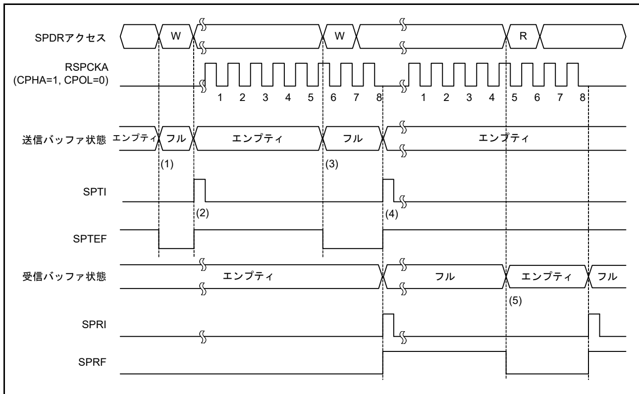
図 32.28 SPTI、SPRI 割り込みの動作例
