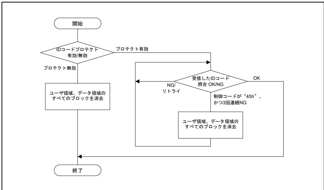
図 41.27 ブートモード ID コードプロテクトの認証フロー
