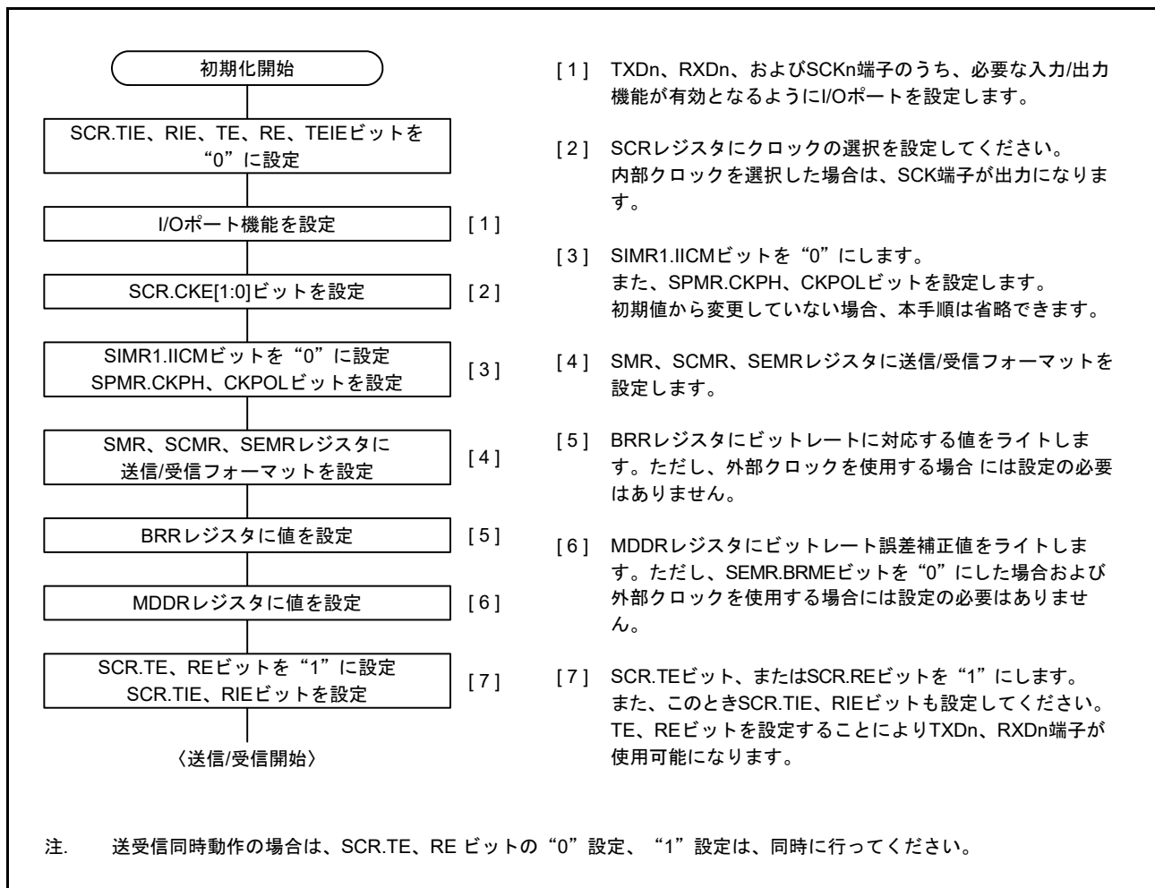
図 29.24 SCIの初期化フローチャートの例(クロック同期式モード)
