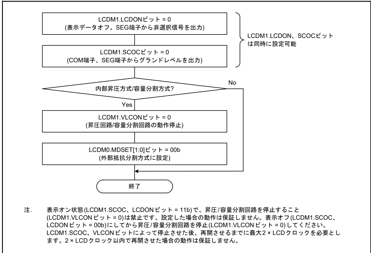
図 34.8 動作停止手順
