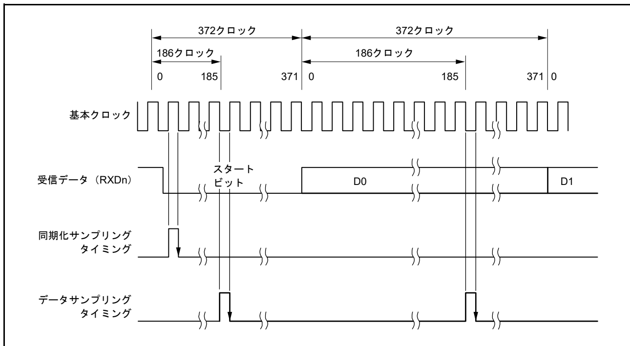
図 29.37 スマートカードインタフェースモード時の受信データサンプリングタイミング (372 倍のクロック使用時)
