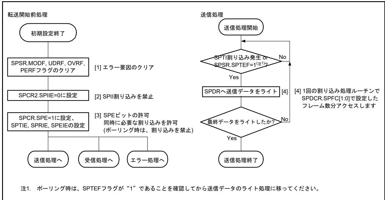
図 32.42 スレーブモード時のフローチャート (送信)
