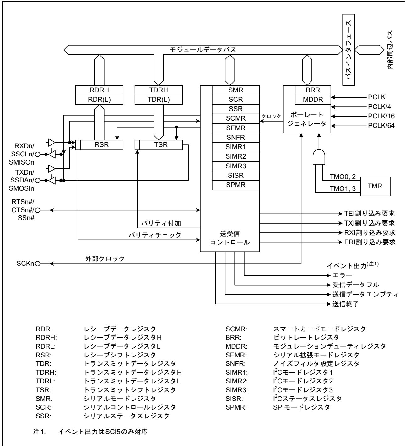
図 29.2 SCIg (SCI5, SCI6) のブロック図
