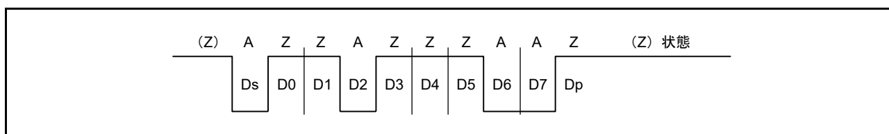
図 29.35 ダイレクトコンベンション (SCMR.SDIR ビット = 0、SCMR.SINV ビット = 0、SMR.PM ビット = 0)
