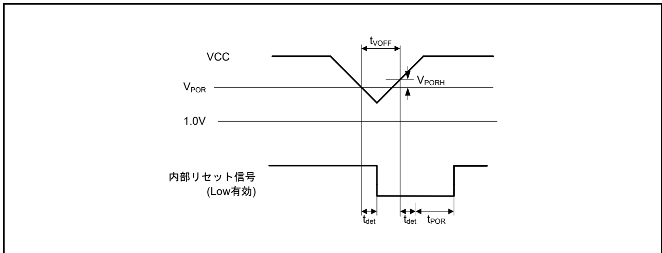
図 42.51 電圧検出リセットタイミング
