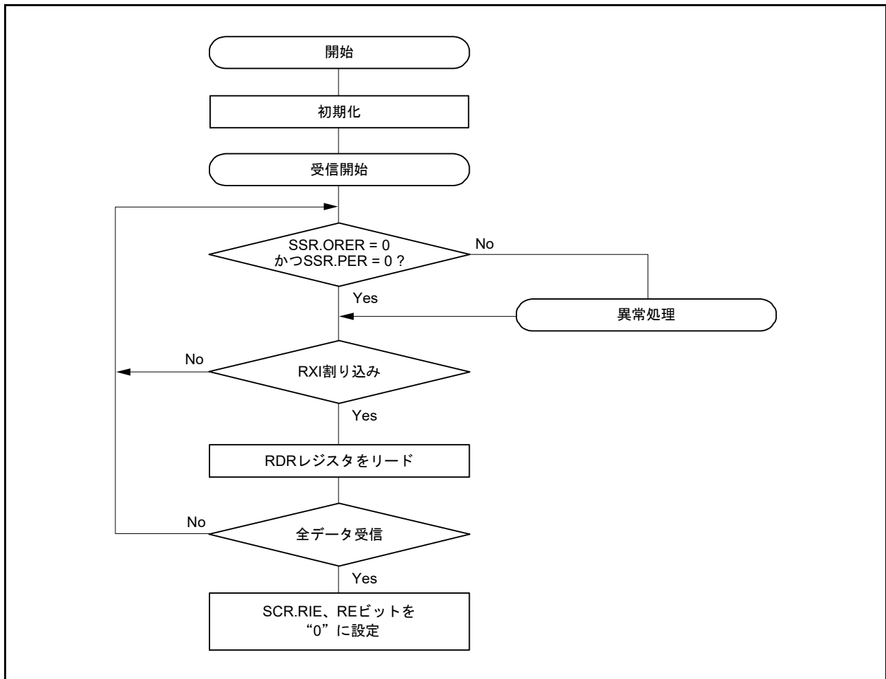
図 29.44 スマートカードインタフェース受信のフローチャート例
