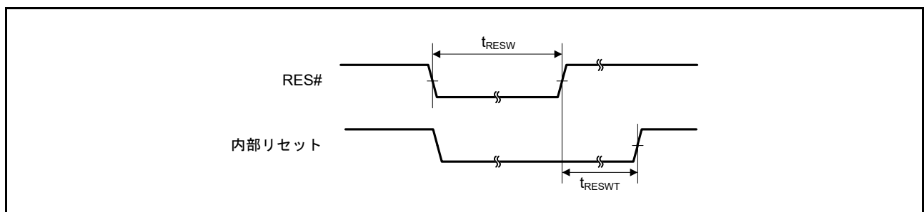
図 42.25 リセット入カタイミング (1)
