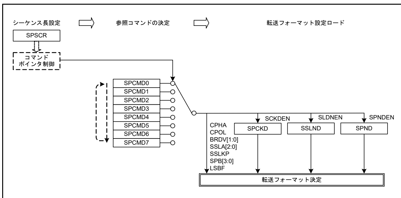
図 32.33 マスタモードでのシリアル転送方式の決定方法
