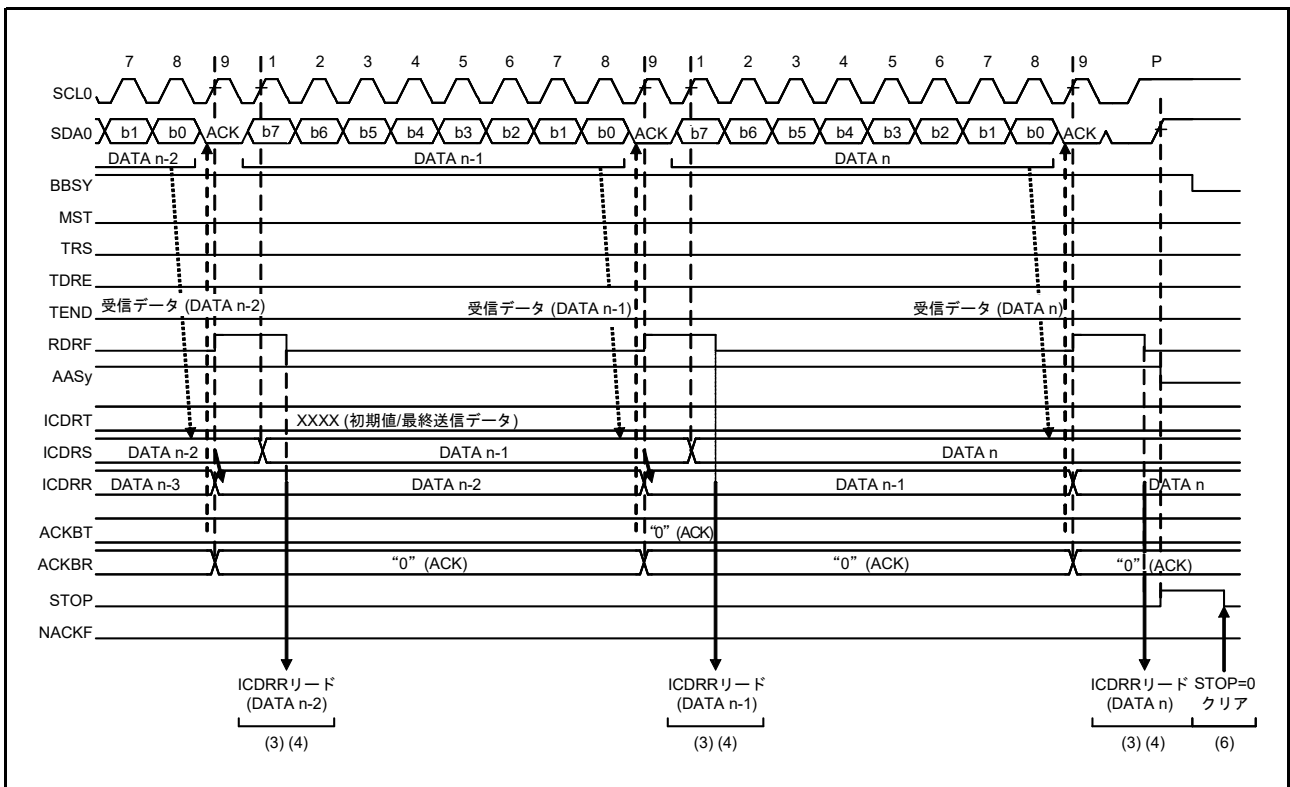
図 30.19 スレーブ受信の動作タイミング (2) (RDRFS ビット = 0 のとき)
