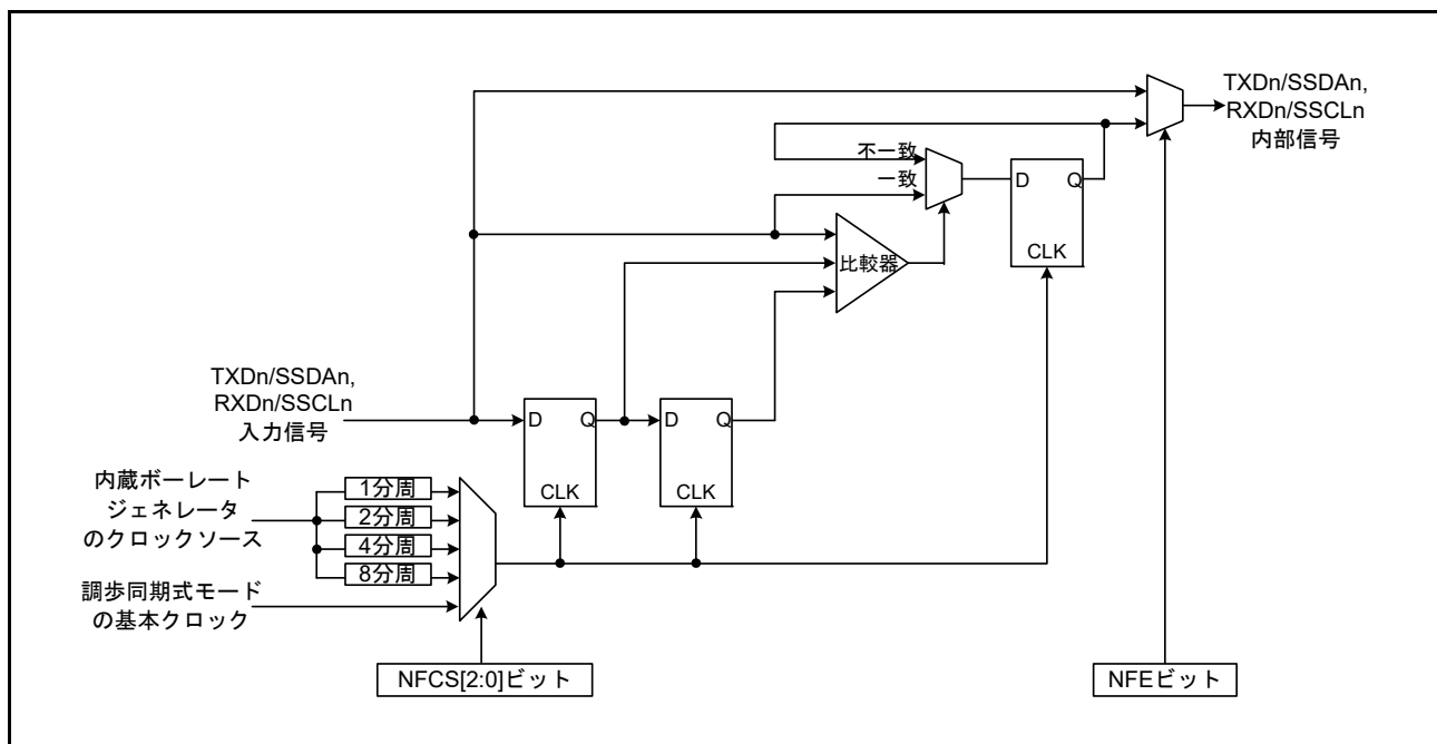
図 29.75 デジタルノイズフィルタのブロック図
