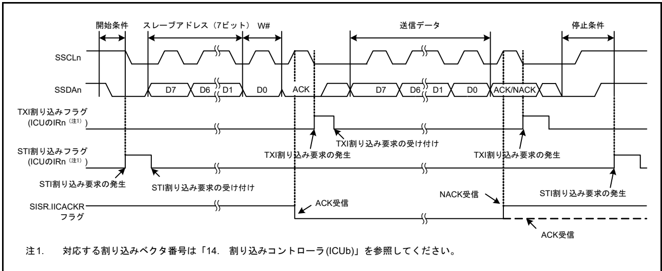
図 29.52 簡易 I 2 C バスモードのマスタ送信の動作例 1 (7 ビットスレーブアドレス、送信割り込み、受信割り込み使用時)
