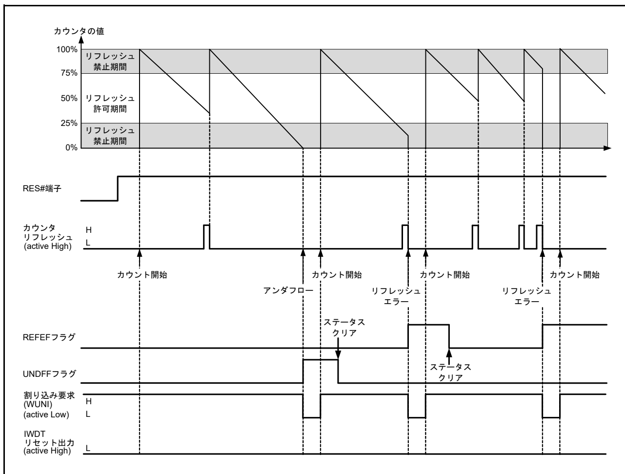
図 28.4 オートスタートモード動作例
