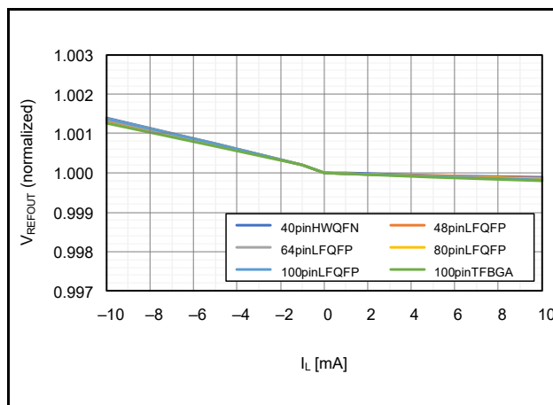
図 42.85 基準電圧源ロードレギュレーション (AVCC0 = 5V, T_a = 25^\circ\text{C} )
