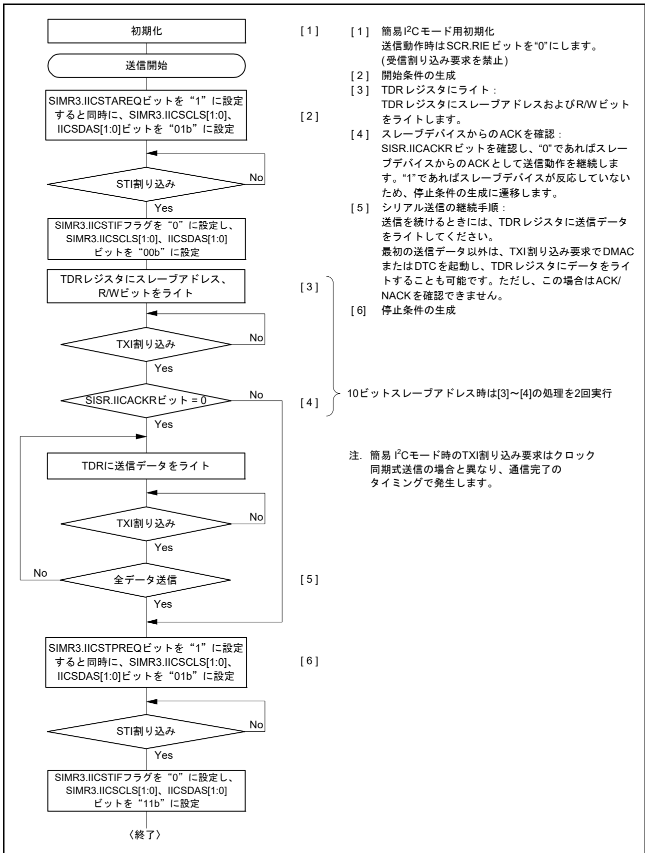
図 29.54 簡易 I 2 C モードのマスタ送信動作のフローチャート例 (送信割り込み、受信割り込み使用時)
