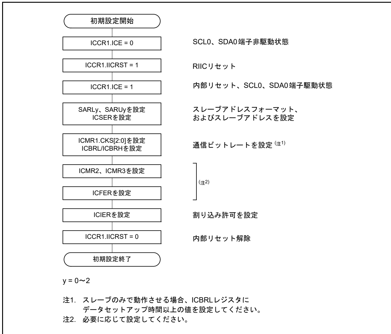
図 30.4 RIIC の初期化フローチャート例
