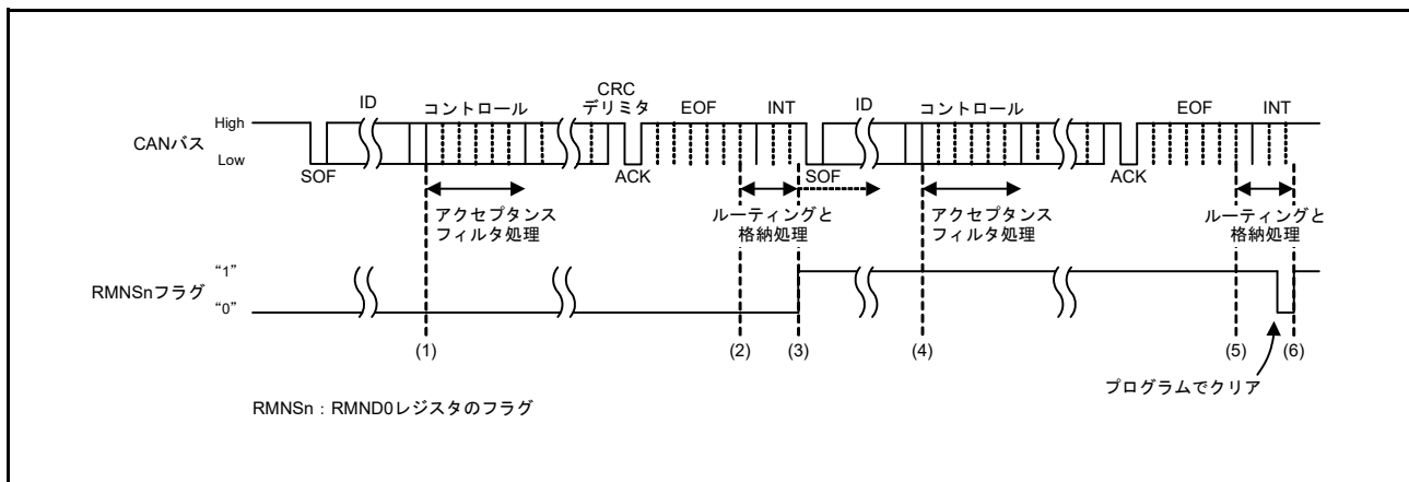
図 31.23 受信バッファの受信タイミング図
