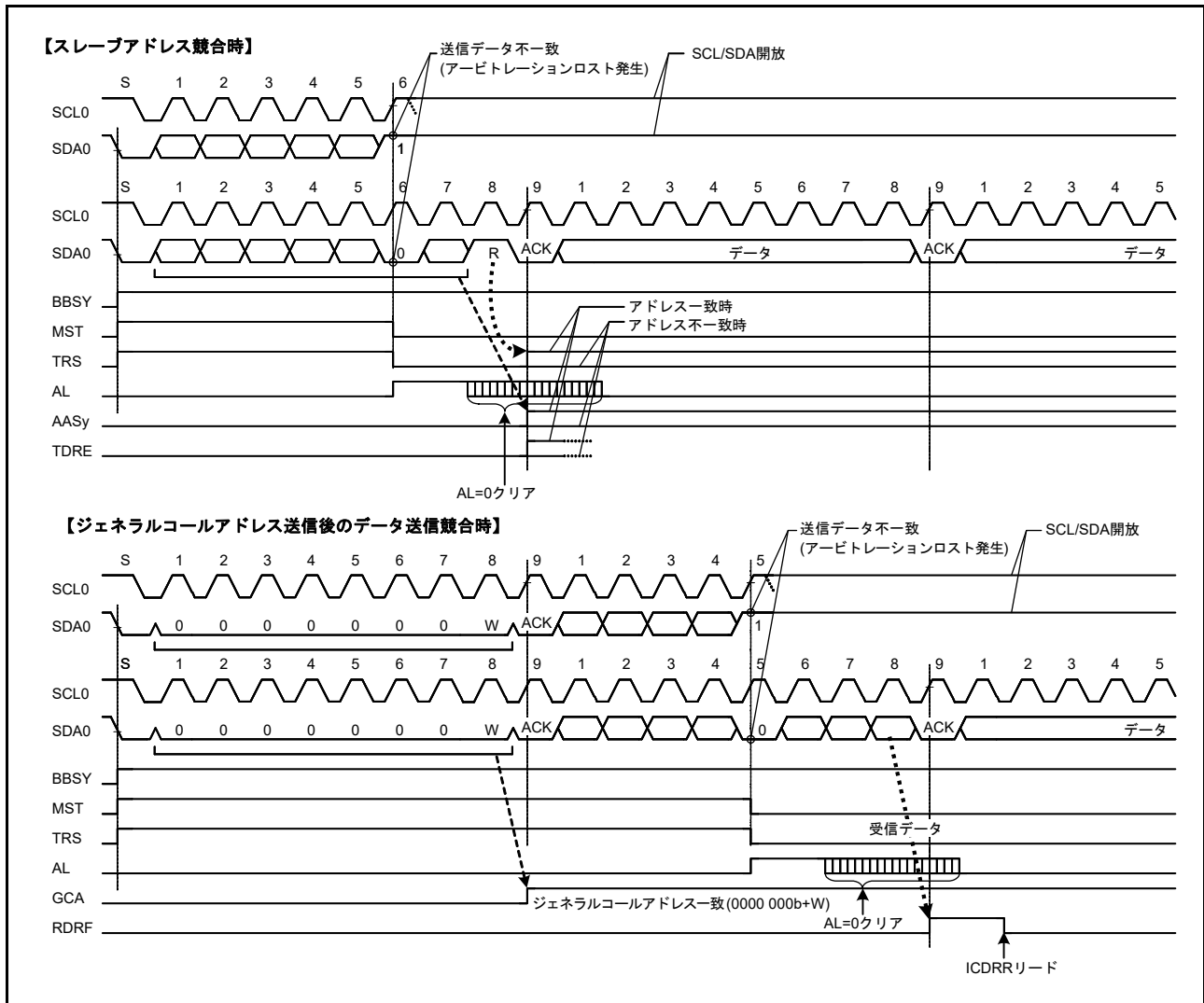
図 30.32 マスタアービトレーションロスト検出動作例 (MALE ビット = 1 のとき)
