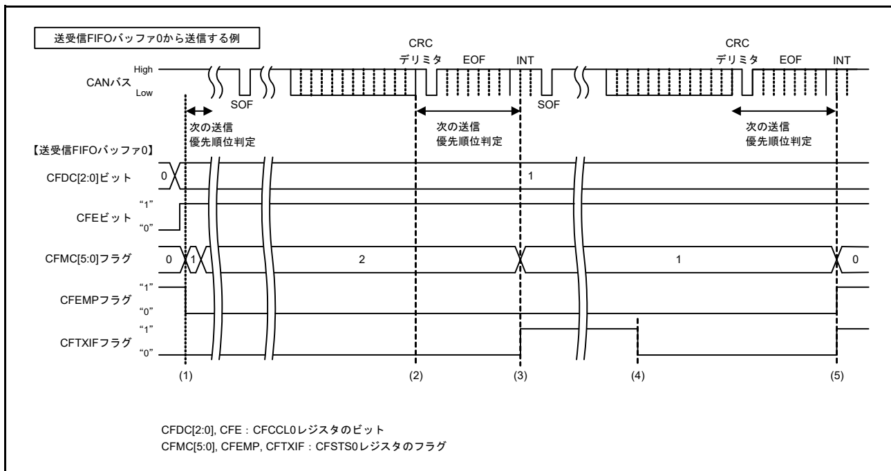
図 31.30 送受信 FIFO バッファの送信タイミング図 (正常に送信完了時)
