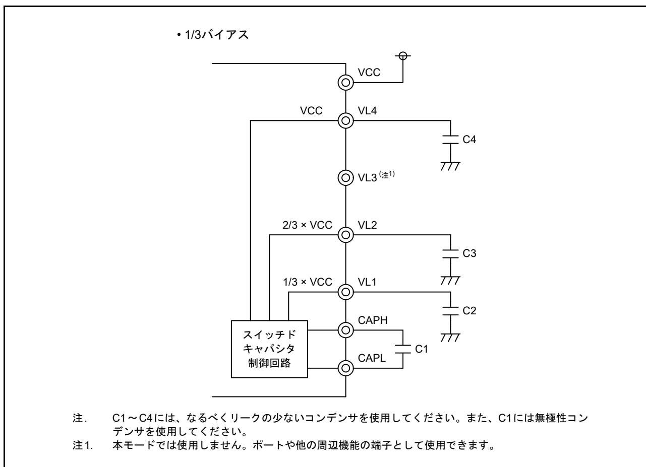
図 34.12 LCD バイアス電圧生成回路の外付け回路例 (容量分割方式)
