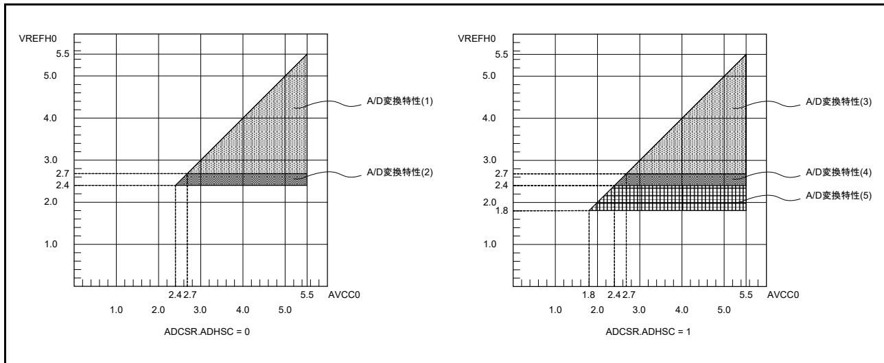
図 42.94 AVCC0-VREFH0 電圧範囲
