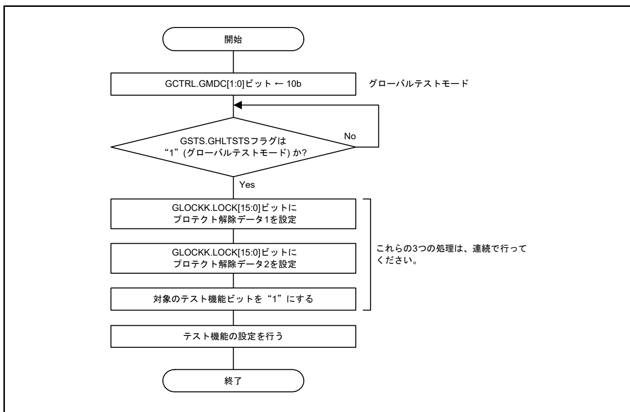
図 31.34 プロテクト解除手順
