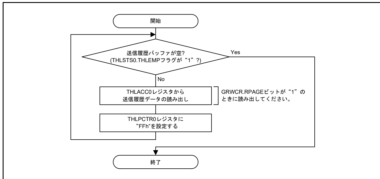
図 31.32 送信履歴バッファの読み出し手順
