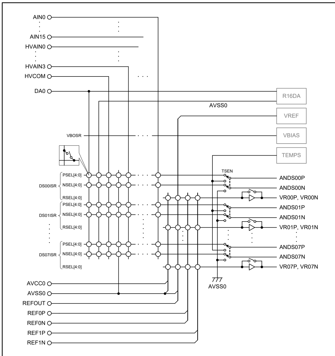
図 35.2 AMUX のブロック図
