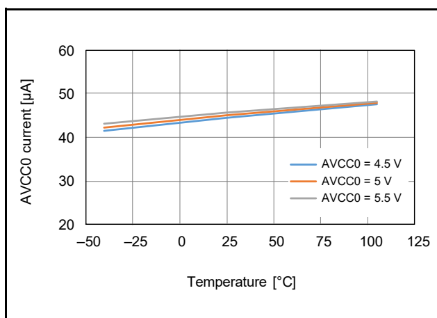
図 42.9 基準電圧源動作電流の温度依存性
