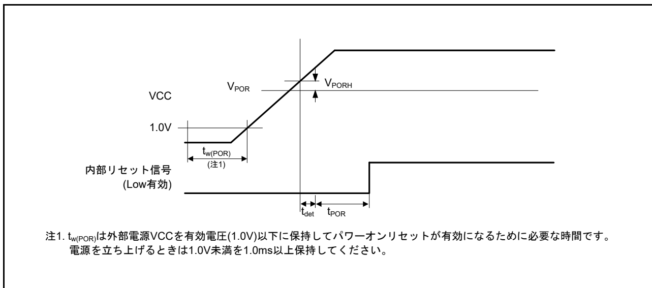
図 42.52 パワーオンリセットタイミング
