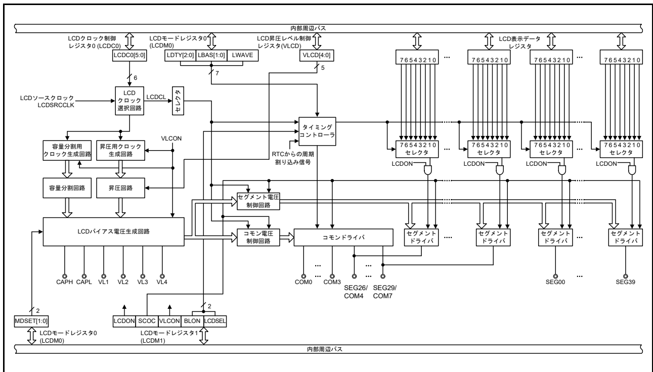
図 34.1 LCDC のブロック図
