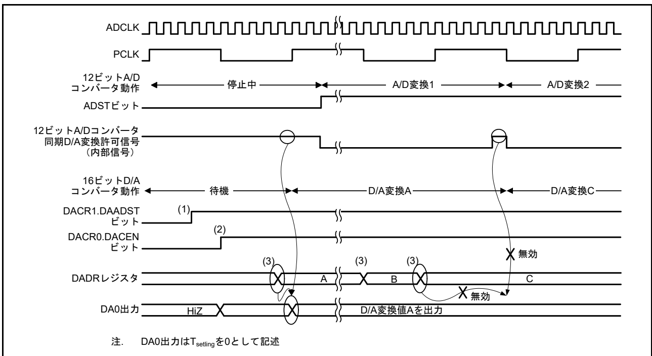
図 38.4 16ビットD/Aコンバータが12ビットA/Dコンバータ同期D/A変換許可信号を取り込めない例
