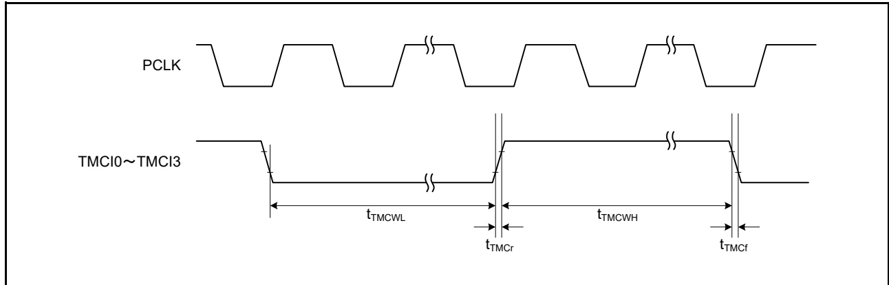
図 42.39 TMR クロック入力タイミング
