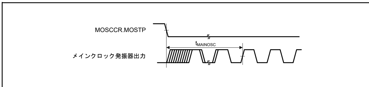
図 42.17 メインクロック発振開始タイミング
