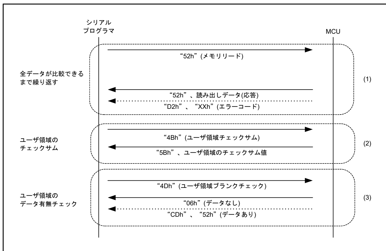
図 41.37 ユーザ領域のデータ確認手順
