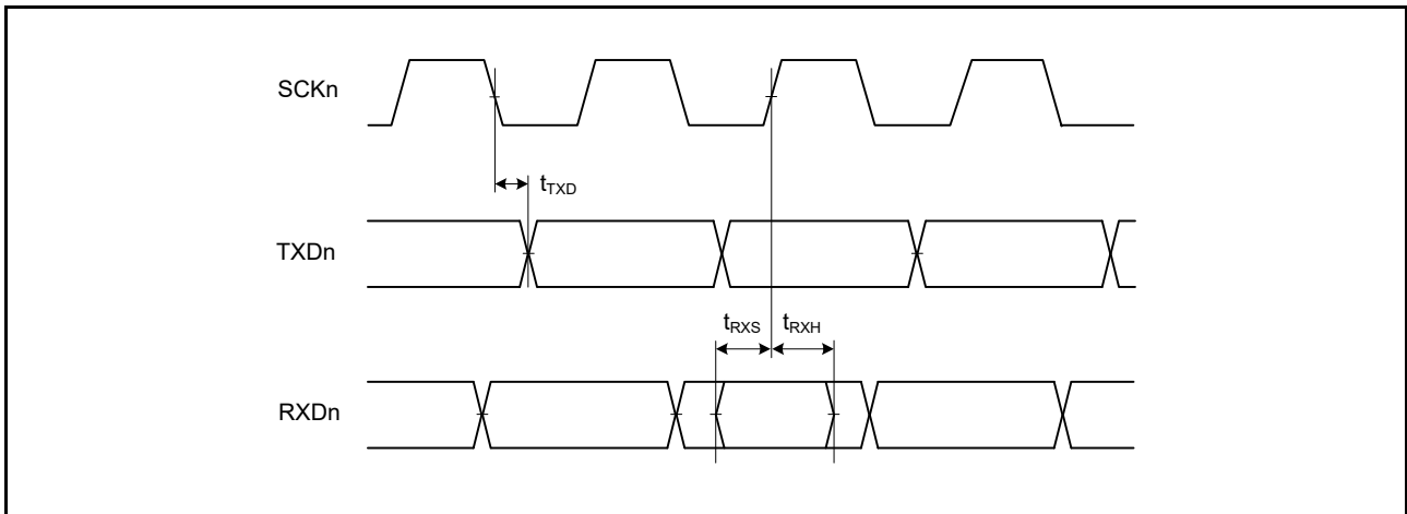
図 42.41 SCI 入出カタイミング / クロック同期式モード (n = 0, 1, 5, 6, 8, 9, 12)
