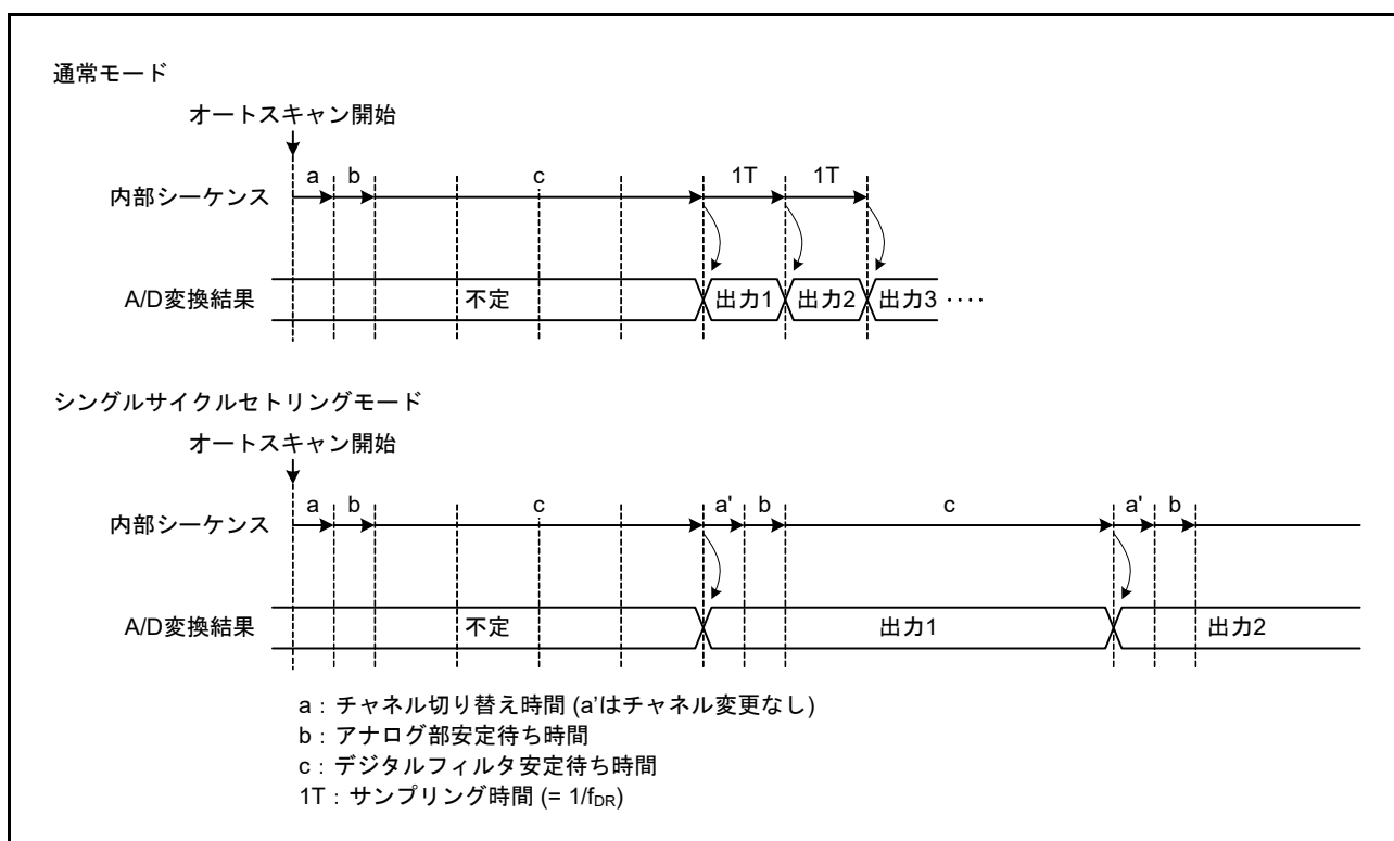
図 36.13 A/D 変換動作モードシーケンス
