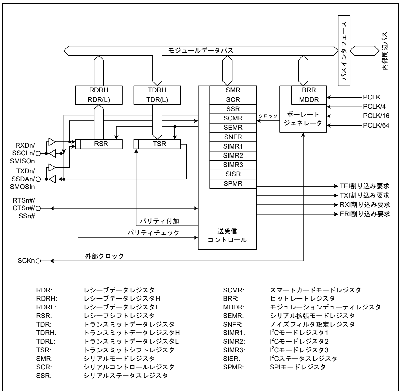
図 29.1 SCIg (SCI0, SCI1, SCI8, SCI9) のブロック図
