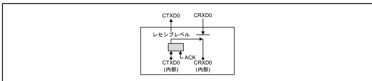
図 31.12 セルフテストモード 1 選択時の接続
