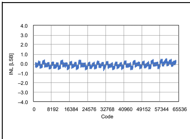
図 42.97 積分非直線性誤差のコード依存性 (AVCC0 = 5V, VREFH = 5V, T_a = 25^\circ\text{C} )
