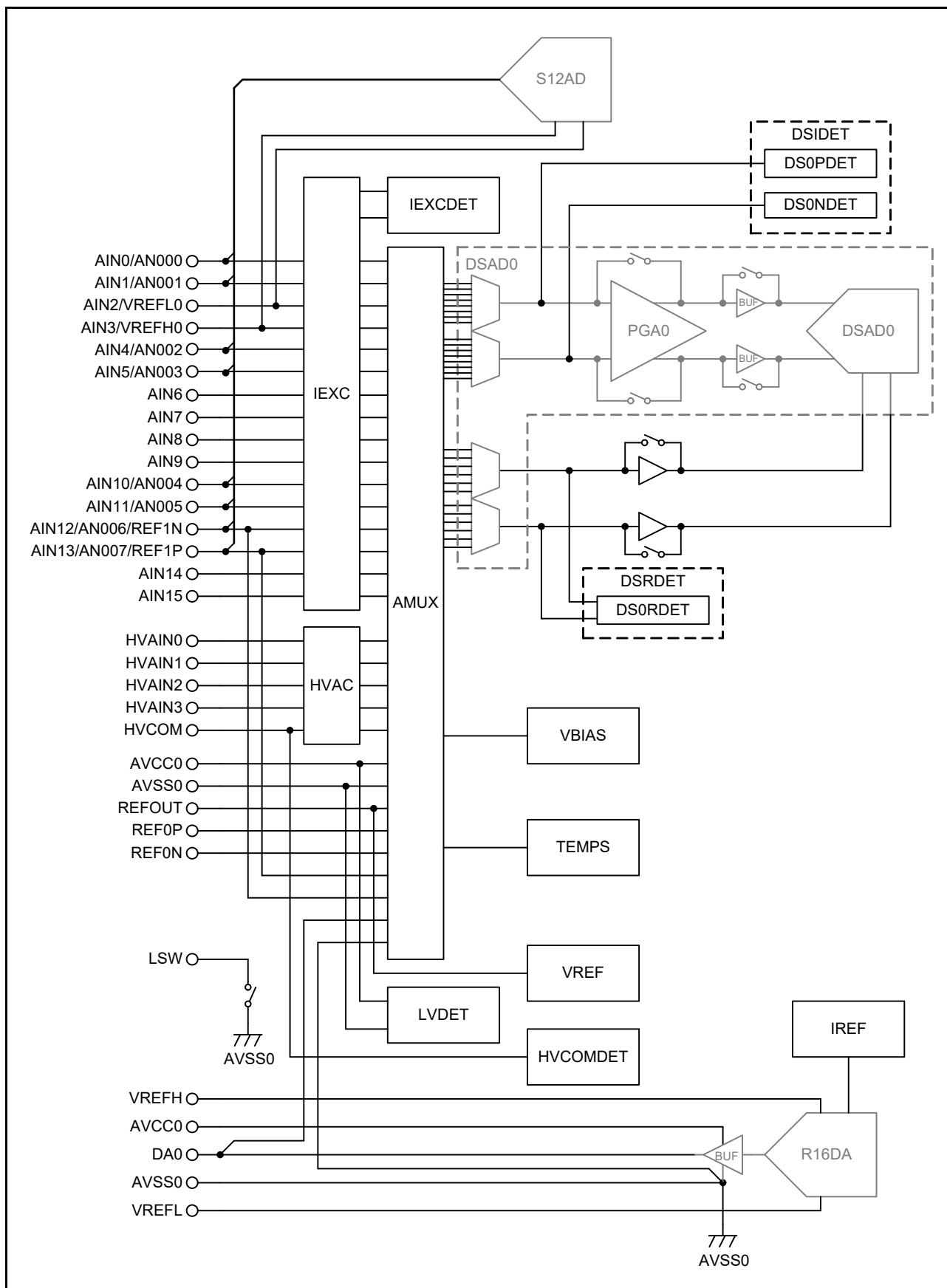
図 35.1 AFE のブロック図
