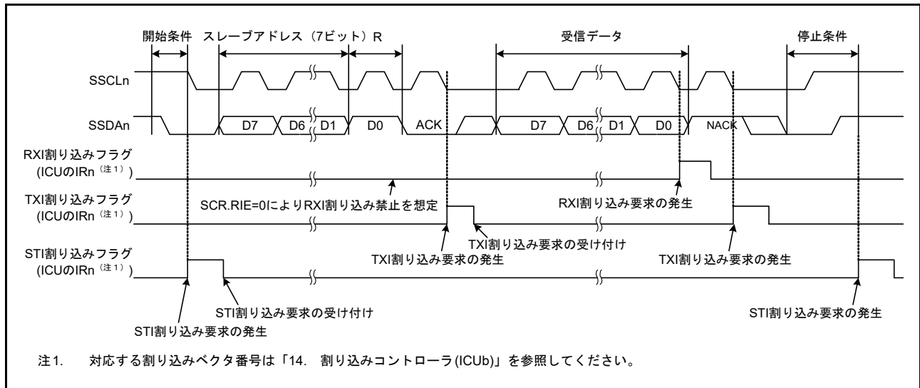
図 29.55 簡易 I 2 C バスモードのマスタ受信の動作例 (7ビットスレーブアドレス、送信割り込み、受信割り込み使用時)
