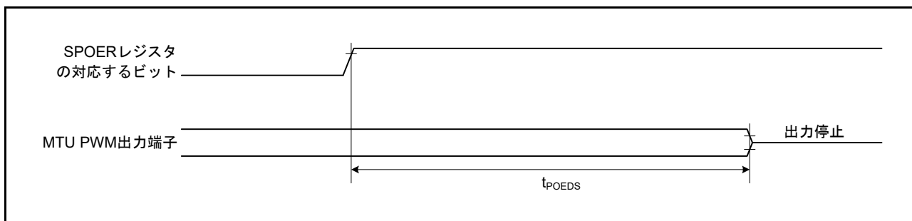
図 42.37 POE 出力ディセーブル時間 (レジスタ設定)
