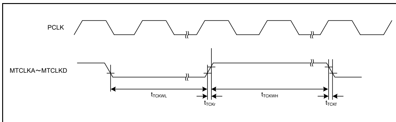
図 42.33 MTU クロック入力タイミング
