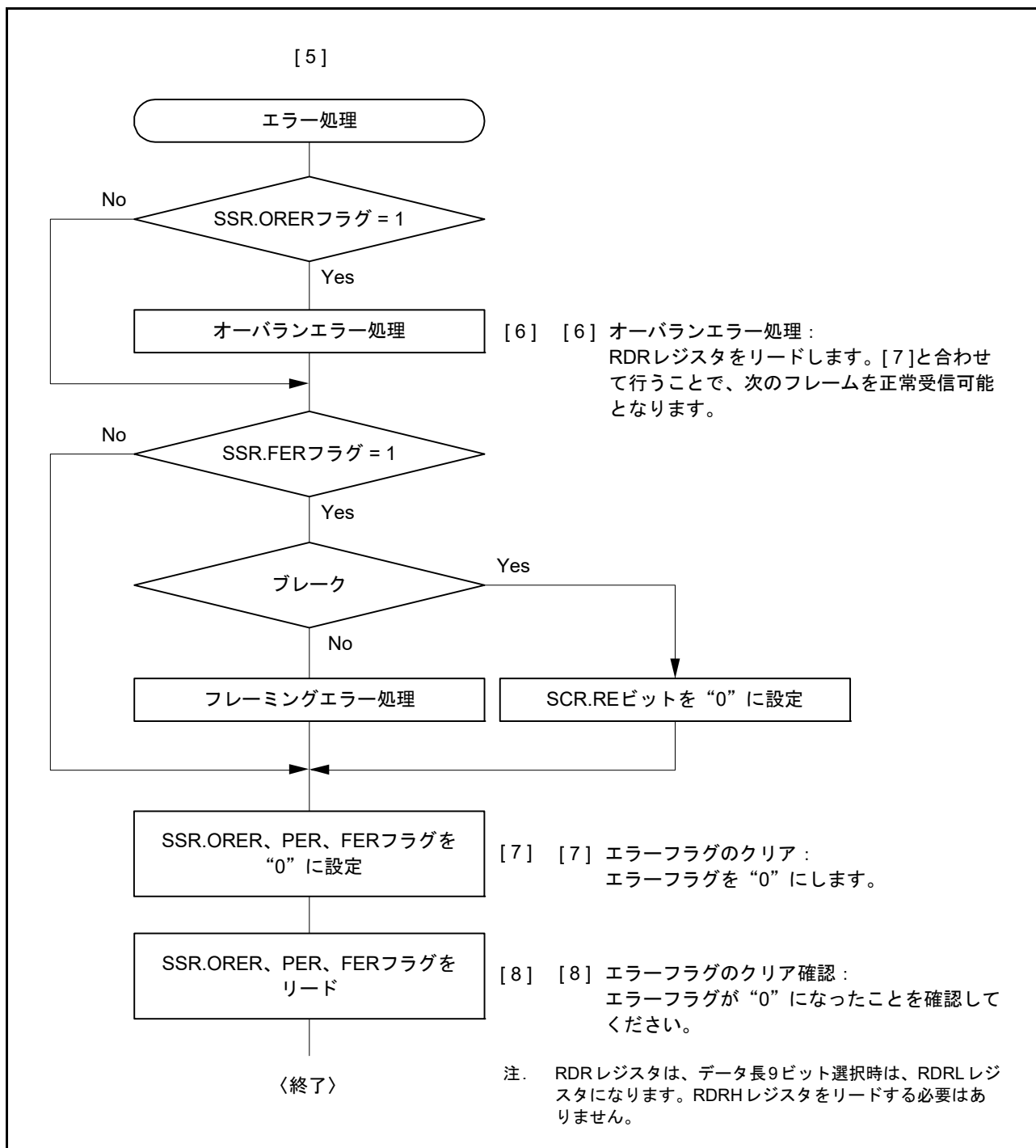
図 29.22 マルチプロセッサシリアル受信のフローチャートの例 (2)
