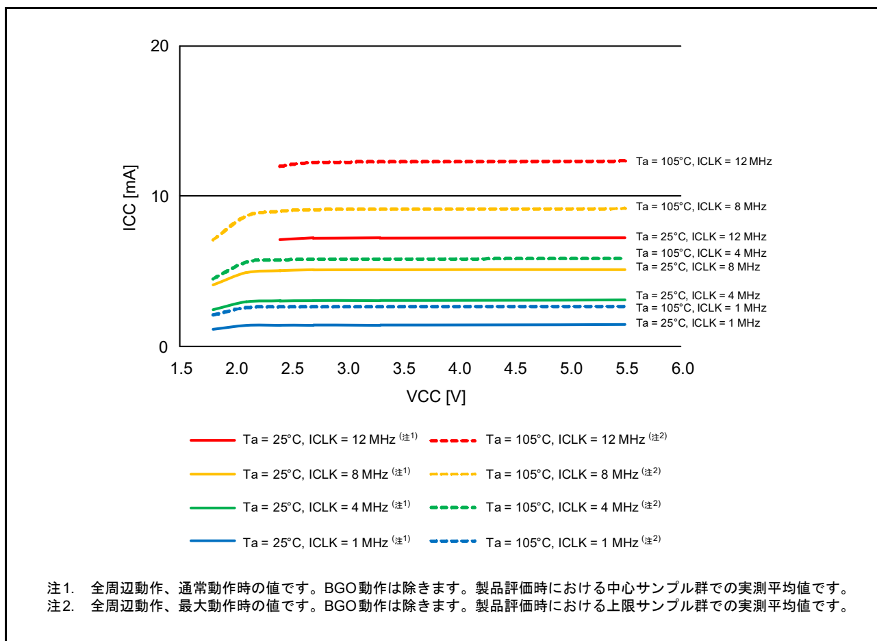
図 42.2 中速動作モードの電圧依存性 (参考データ)
