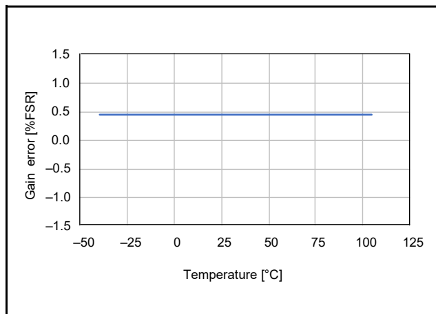
図 42.100 ゲインエラーの温度依存性 (AVCC0 = 5V, VREFH = 5V)
