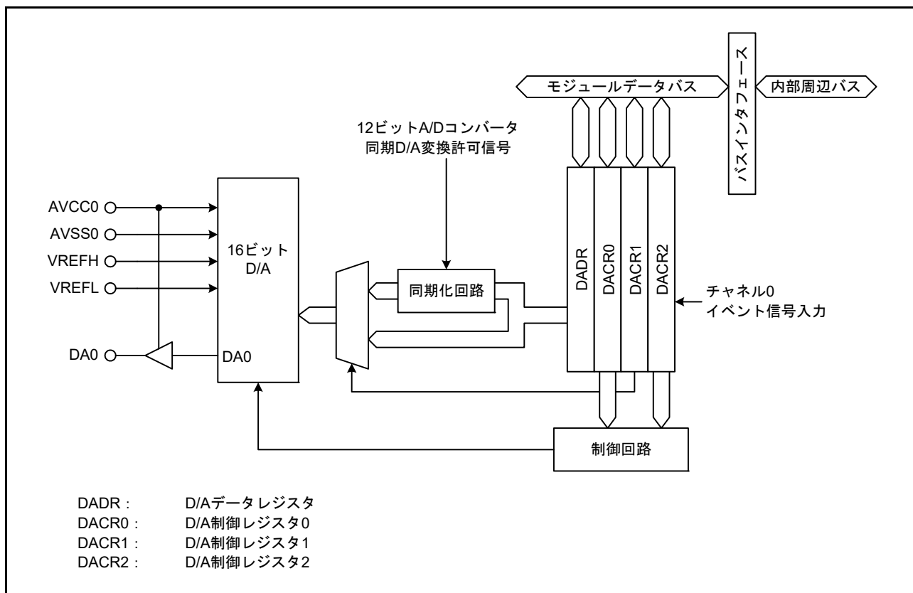
図38.1 16ビットD/Aコンバータのブロック図
