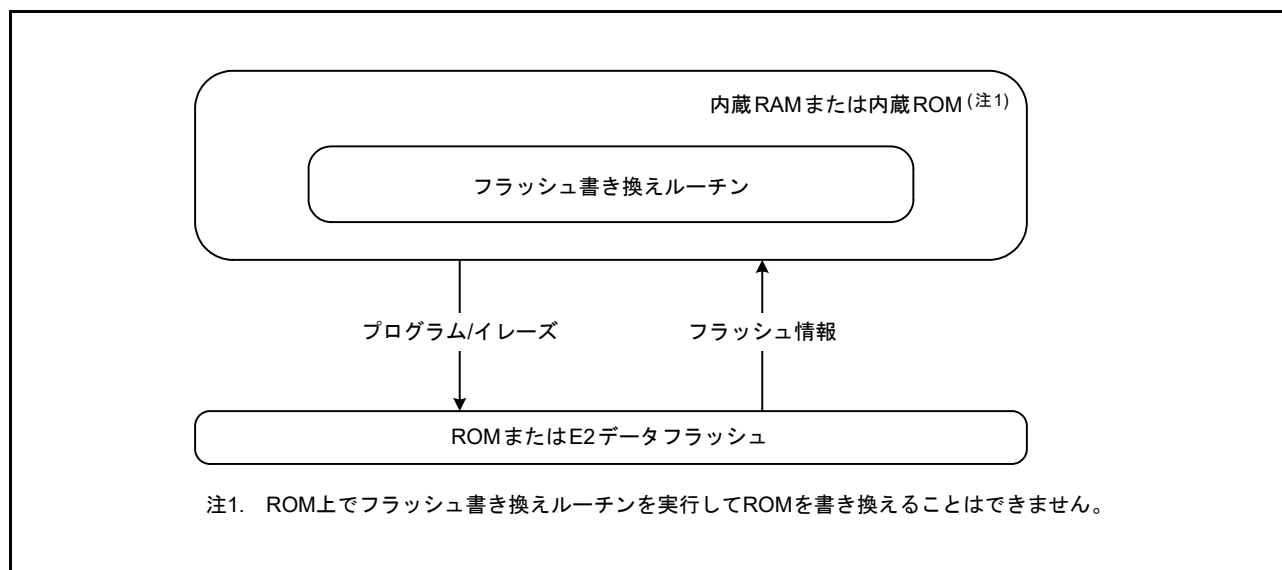
図 41.40 セルフプログラミングの概念
