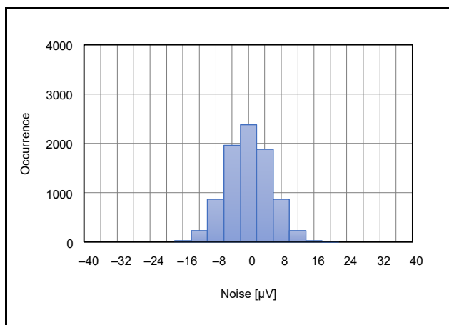
図 42.59 ノイズヒストグラム (AVCC0 = 5.0V、 T_a = 25^\circ\text{C} 、Gain = 64、 f_{\text{MOD}} = 4\text{MHz} 、 f_{\text{DR}} = 125\text{k SPS} 、Sinc 5 フィルタ、 V_{\text{ID}} = 0\text{V} 、 V_{\text{REF}} = 2.5\text{V} 、リファレンスバッファ無効)
