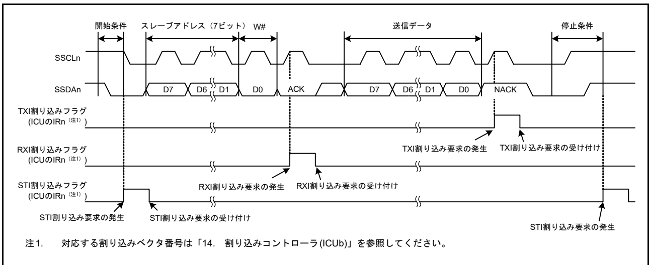
図 29.53 簡易 I 2 C バスモードのマスタ送信の動作例 2 (7 ビットスレーブアドレス、ACK 割り込み、NACK 割り込み使用時)
