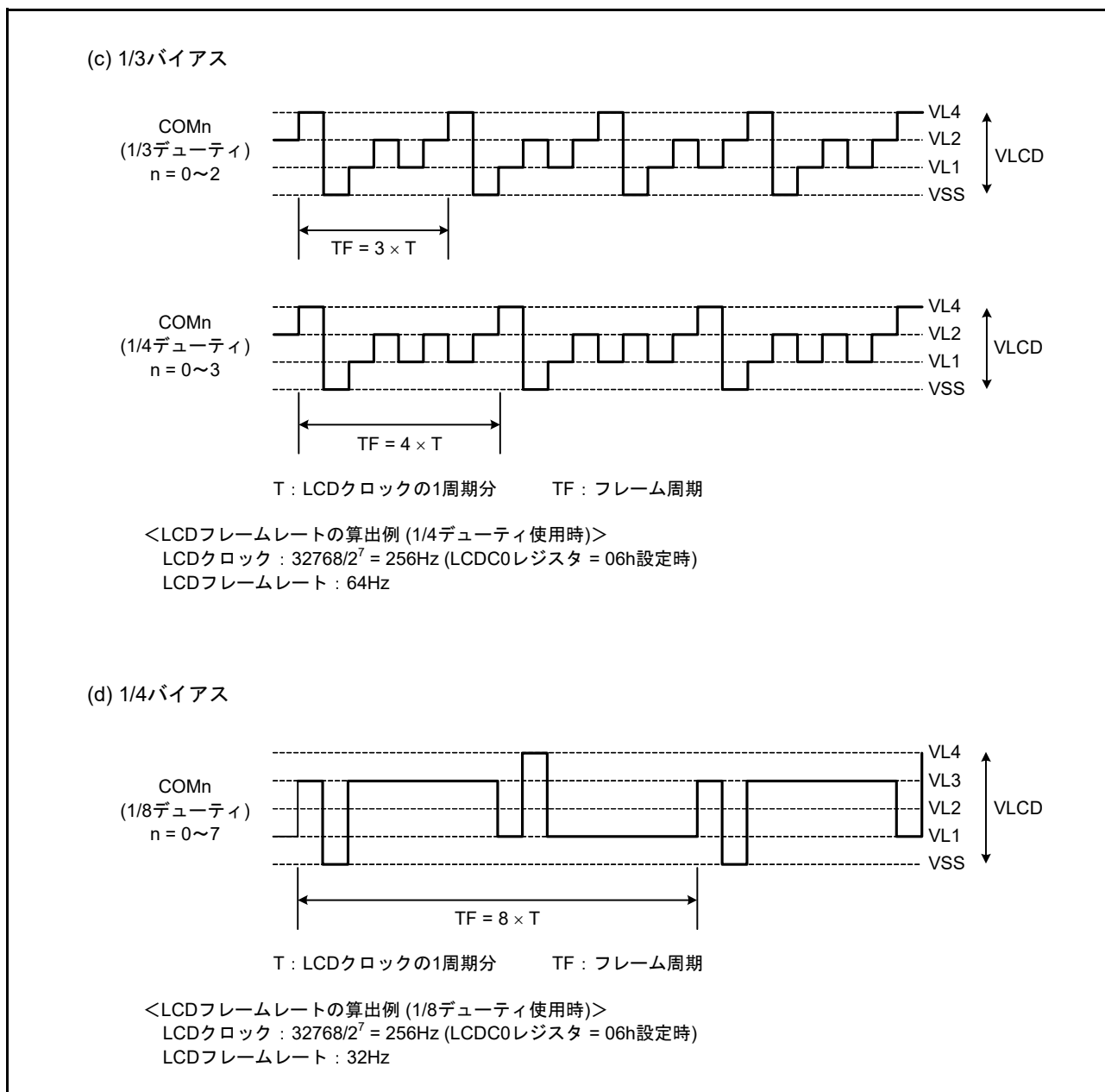
図 34.14 コモン信号波形 (2)
