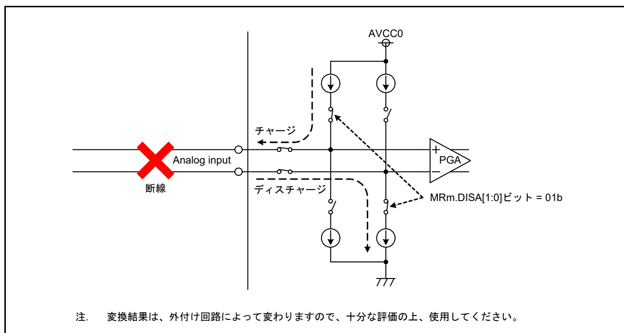
図 36.14 断線検出の例
