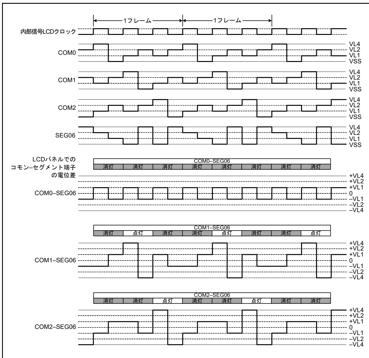
図 34.27 SEG06 端子と各コモン端子間の 1/3 デューティ LCD 駆動波形例 (1/3 バイアス)
