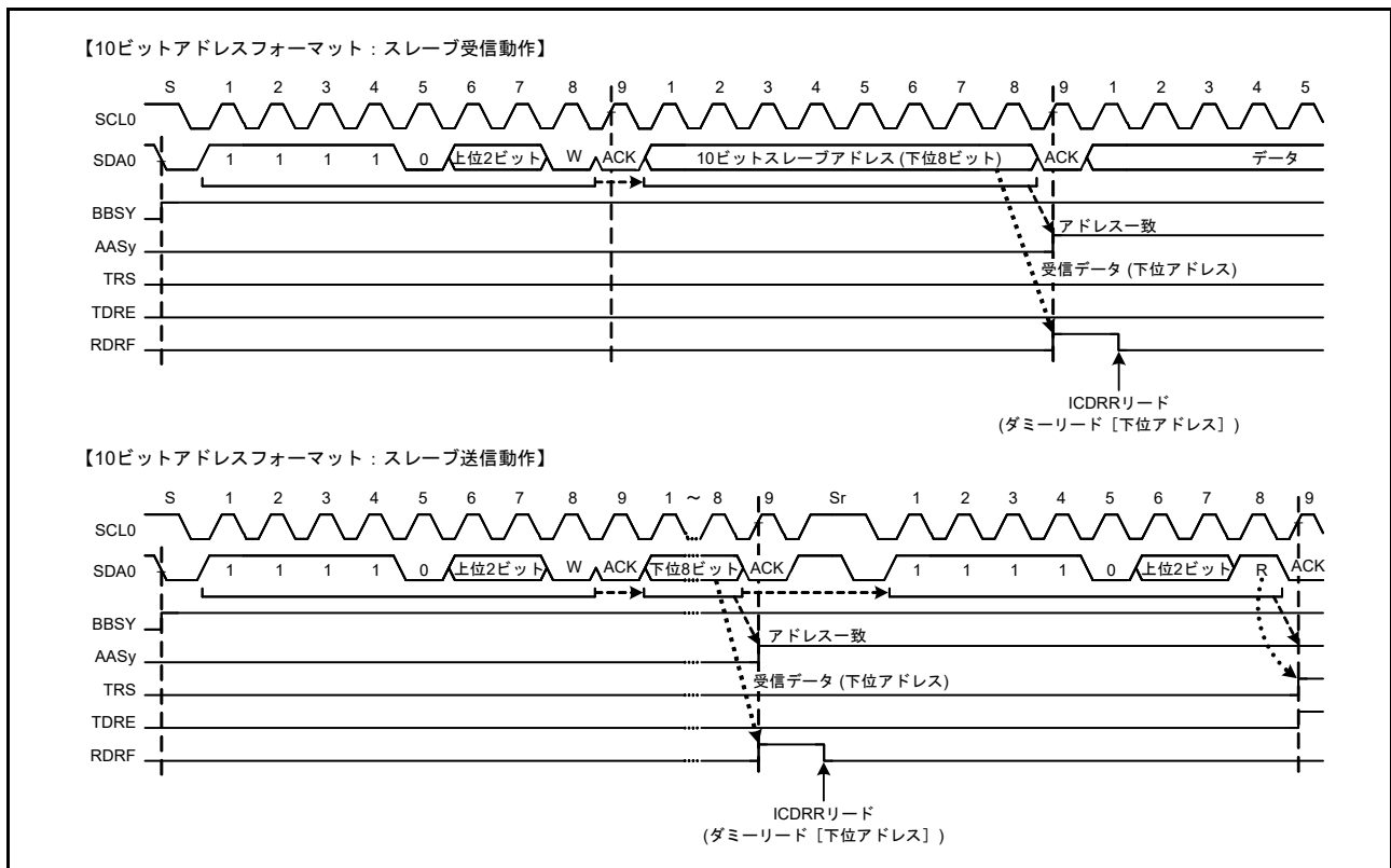
図 30.24 10ビットアドレスフォーマット選択時にAASyフラグが“1”になるタイミング
