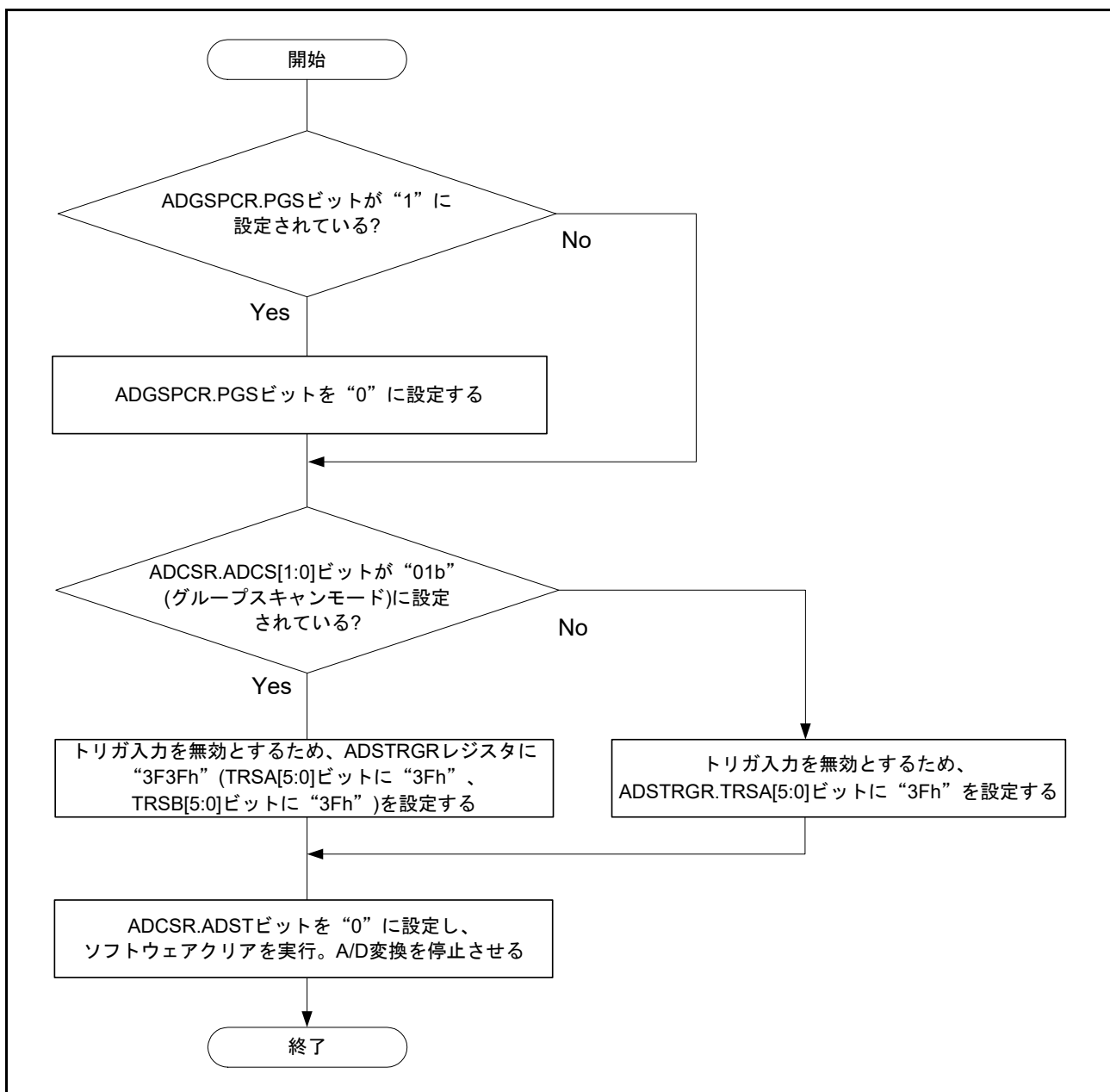
図 37.28 ADCSR.ADST ビットによるソフトウェアクリア実行の設定フロー
