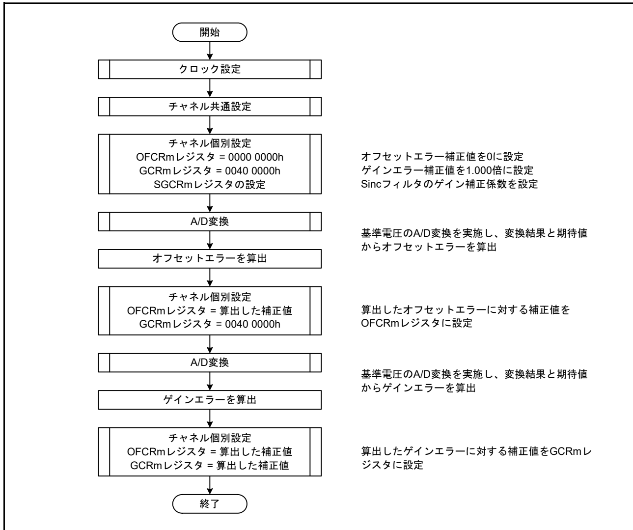
図 36.21 オフセットエラー/ゲインエラー補正値算出フロー (m = 0 ~ 7)
