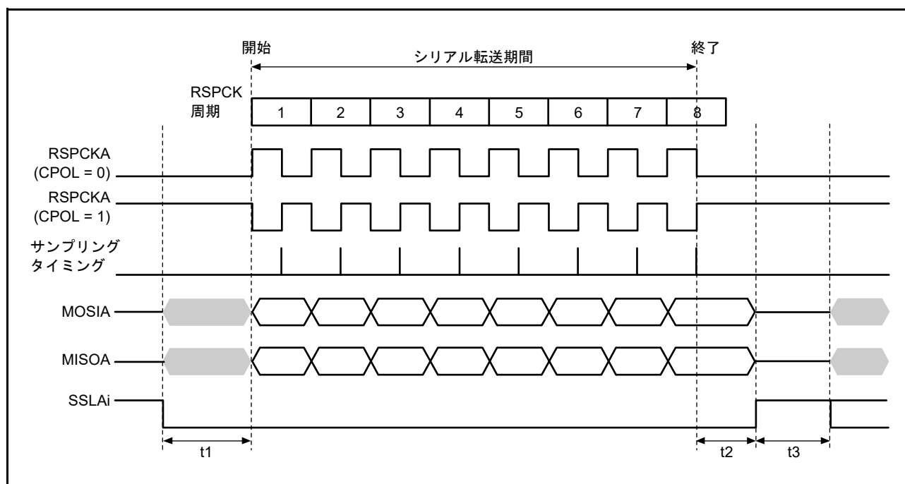
図 32.25 RSPI 転送フォーマット (CPHA ビット = 1)
