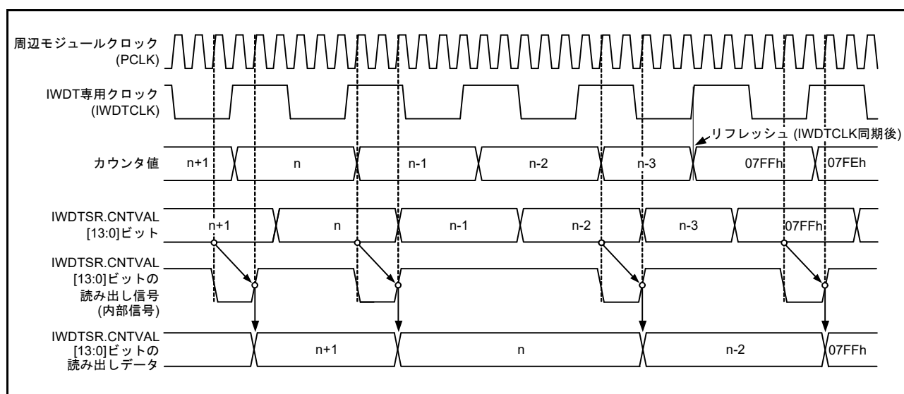
図 28.7 IWDT カウンタ値の読み出し処理 (IWDTCR.CKS[3:0] = 0000b、IWDTCR.TOPS[1:0] = 11b)
