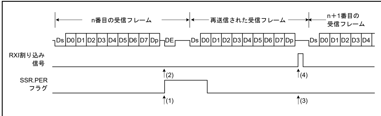
図 29.43 SCI 受信モードの場合の再送信動作 (受信時の再送信動作)
