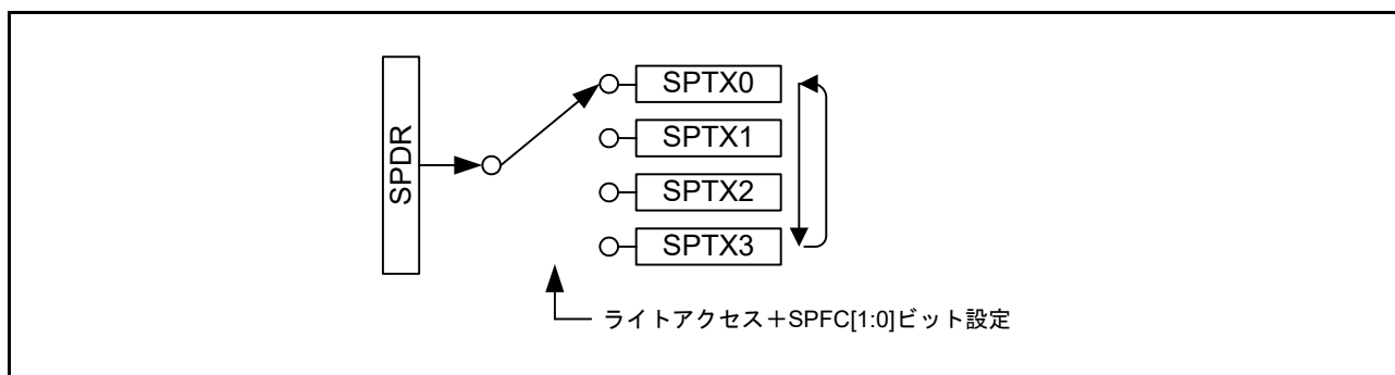
図 32.3 SPDR レジスタの構成図 (ライト時)
