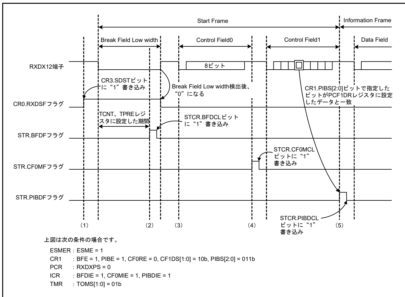
図 29.68 Start Frame の受信時の動作例 (プライオリティインタラプトビット使用時)
