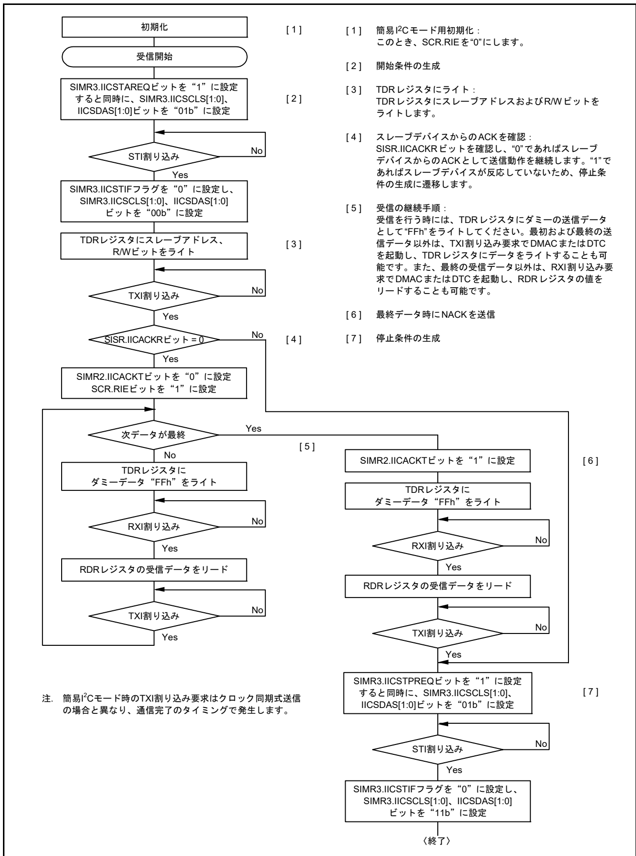
図 29.56 簡易 I 2 C モードのマスタ受信動作のフローチャート例 (送信割り込み、受信割り込み使用時)
