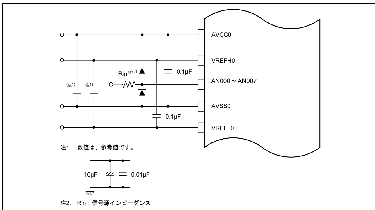
図 37.31 アナログ入力保護回路の例
