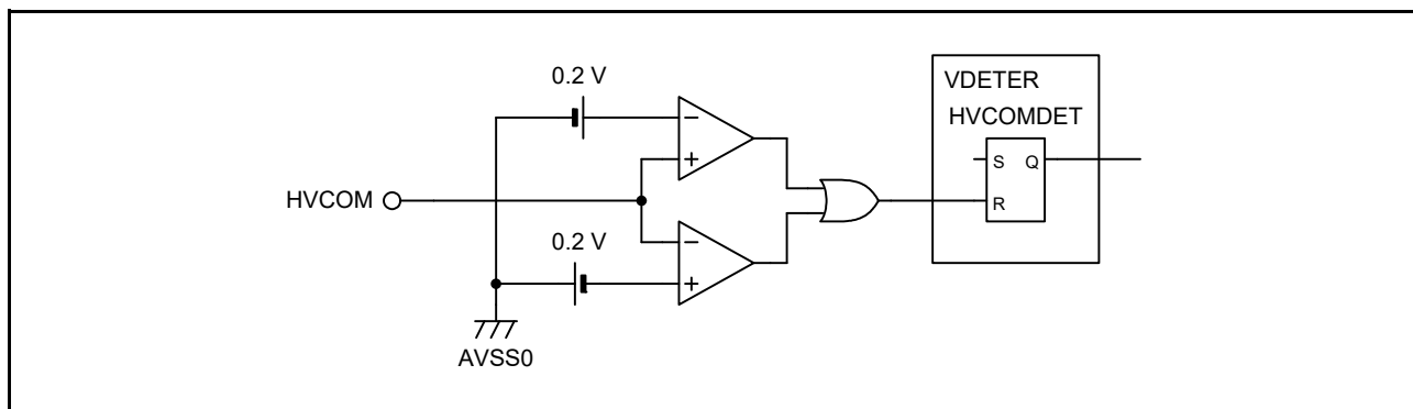
図 35.14 HVCOMDET のブロック図
