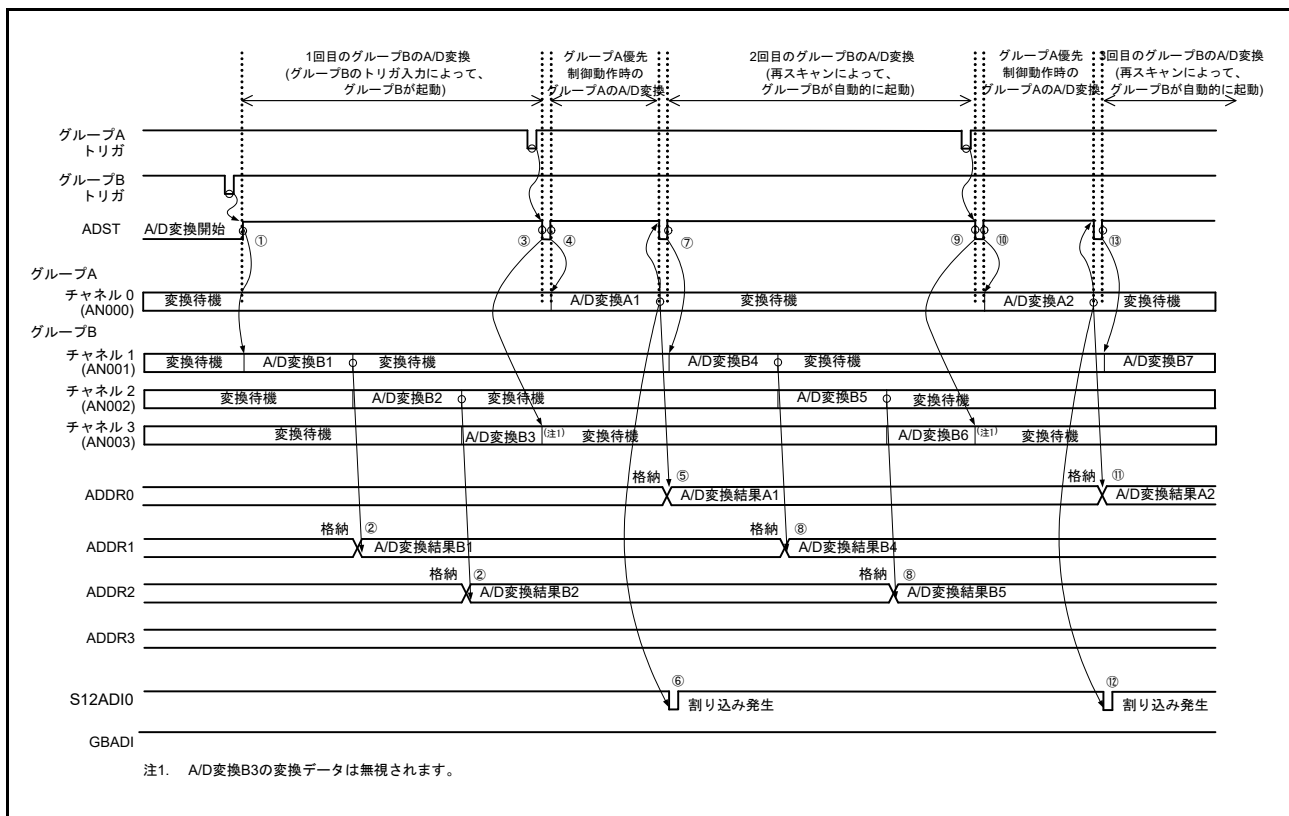
図 37.14 グループ A 優先制御の動作例 (2) (ADGSPCR.GBRSCN = 1、ADGSPCR.GBRP = 0 時の動作)
