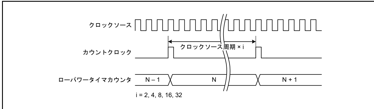
図 27.4 ローパワータイマカウンタのカウンタタイミング
