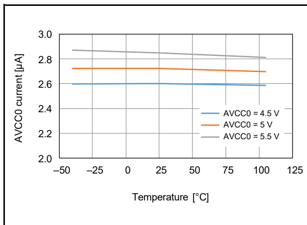
図 42.14 リファレンスバッファ動作電流の温度依存性
