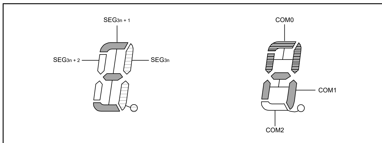
図 34.24 1/3 デューティ LCD の表示パターンと電極結線 (n = 0 ~ 7)
