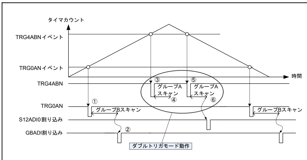
図 37.11 グループスキャンモードでダブルトリガモード選択時の動作例 (MTU からの同期トリガ発生による基本動作)
