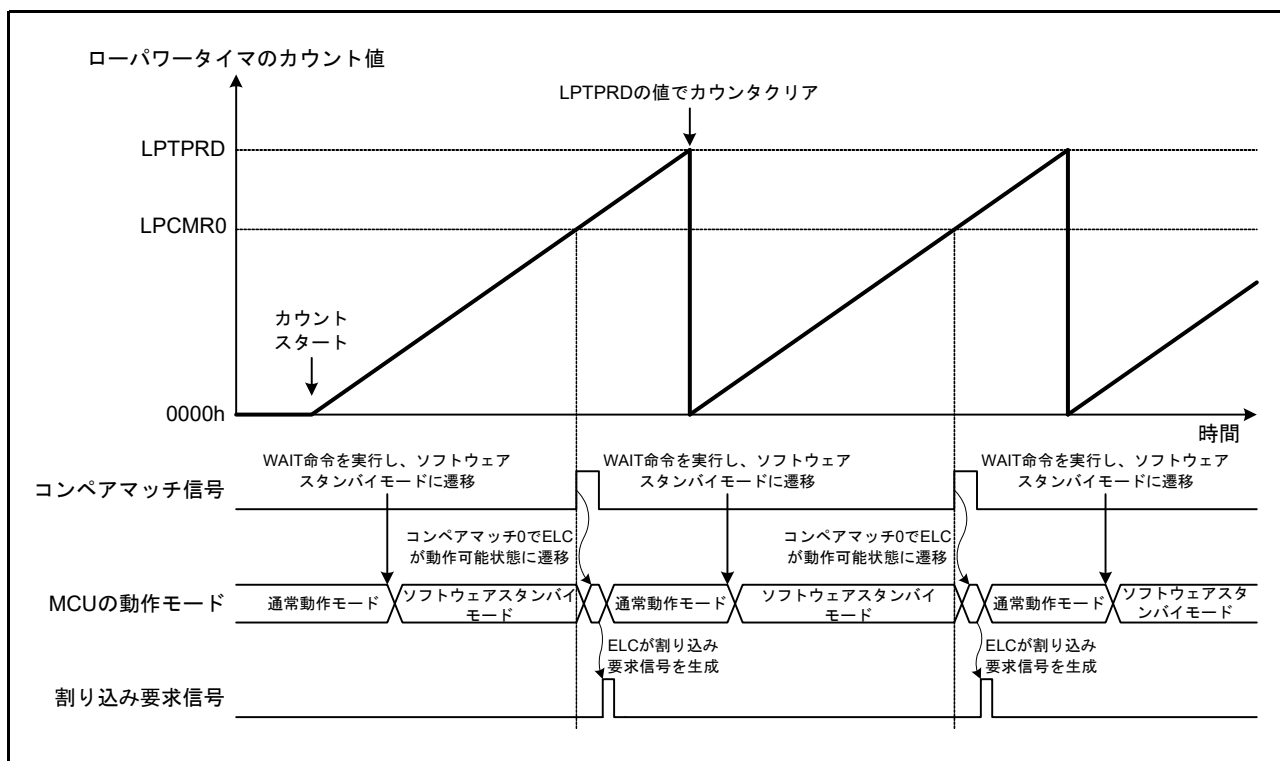
図 27.2 ローパワータイマの動作
