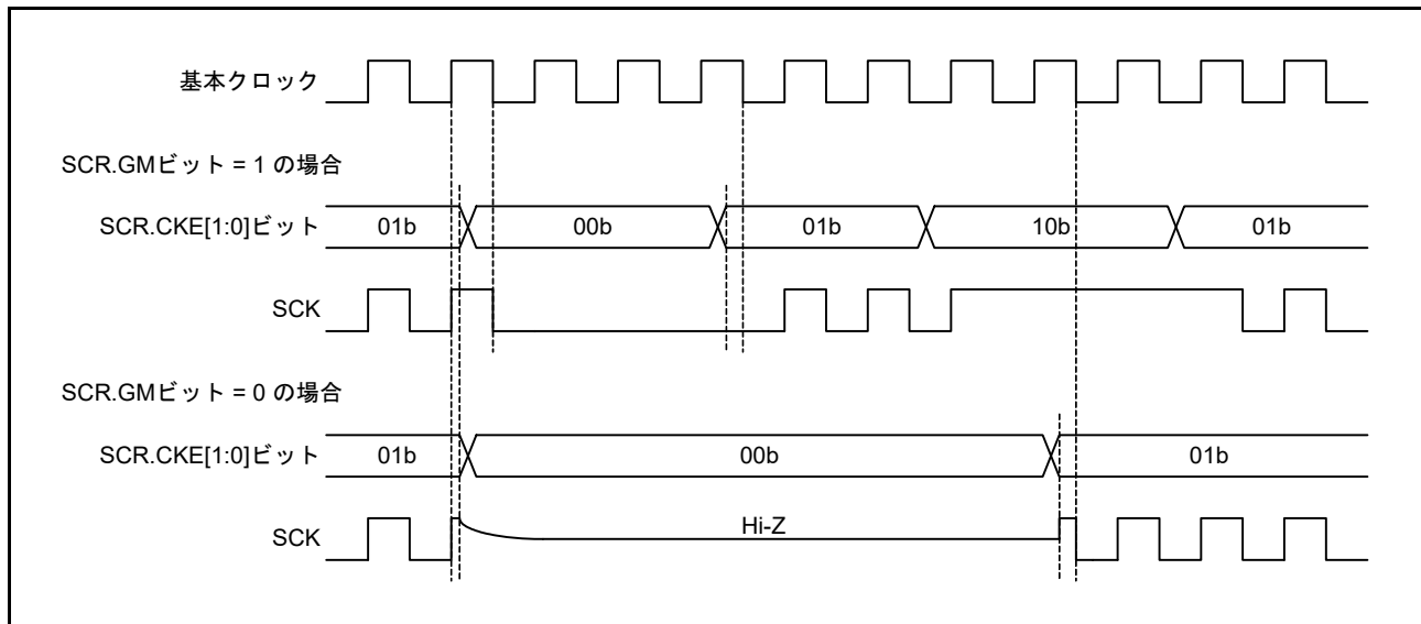
図 29.45 クロック出力制御
