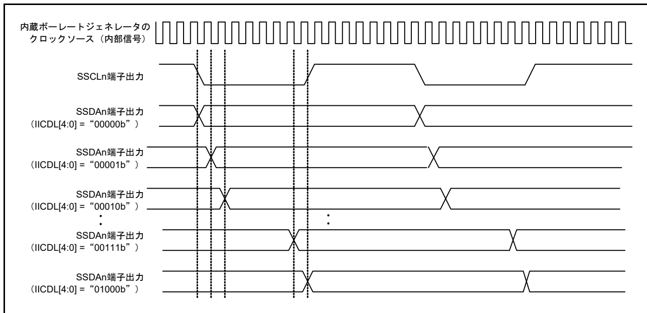
図 29.50 SSDA 出力遅延のタイミング
