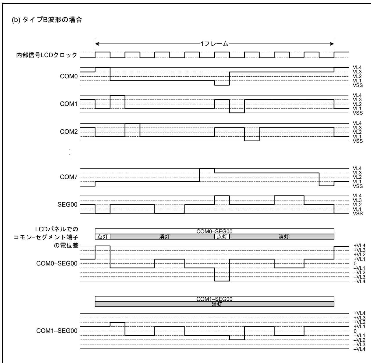
図 34.35 SEG00 端子と各コモン端子間の 1/8 デューティ LCD 駆動波形例 (1/4 バイアス) (2)
