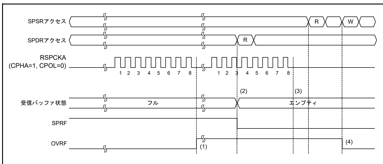
図 32.29 SPRF フラグと OVRF フラグの動作例
