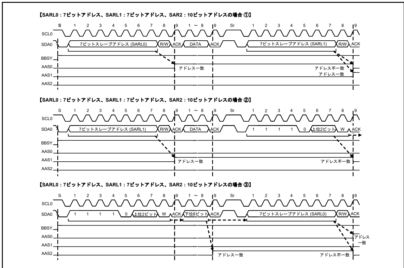
図 30.25 7ビット/10ビットアドレスフォーマット混在時にAASyフラグが“1”または“0”になるタイミング
