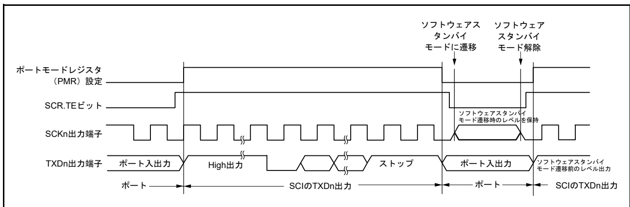
図 29.78 ソフトウェアスタンバイモード遷移時のポートの端子状態 (内部クロック、調歩同期送信)
