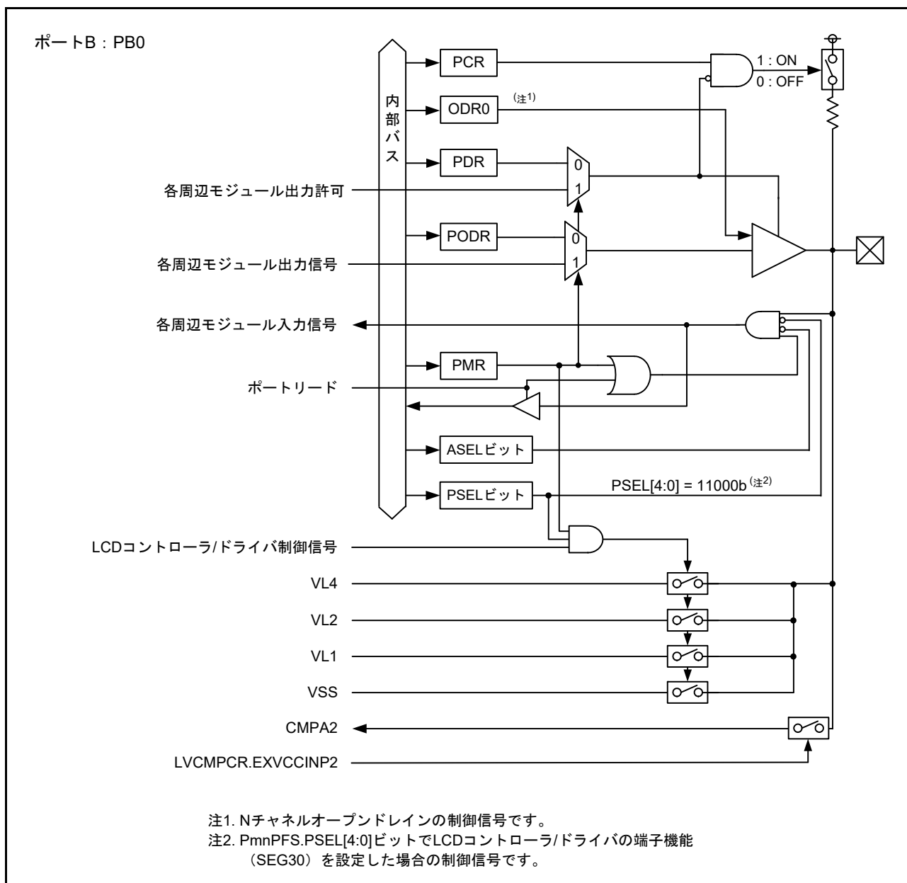
図 20.6 入出力ポートの構成 (6)
