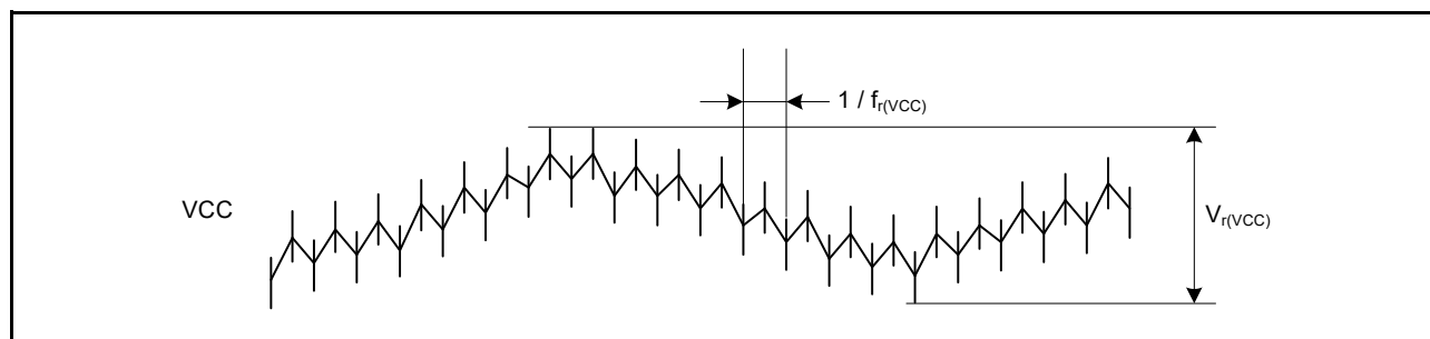
図 42.6 電源リップル波形
