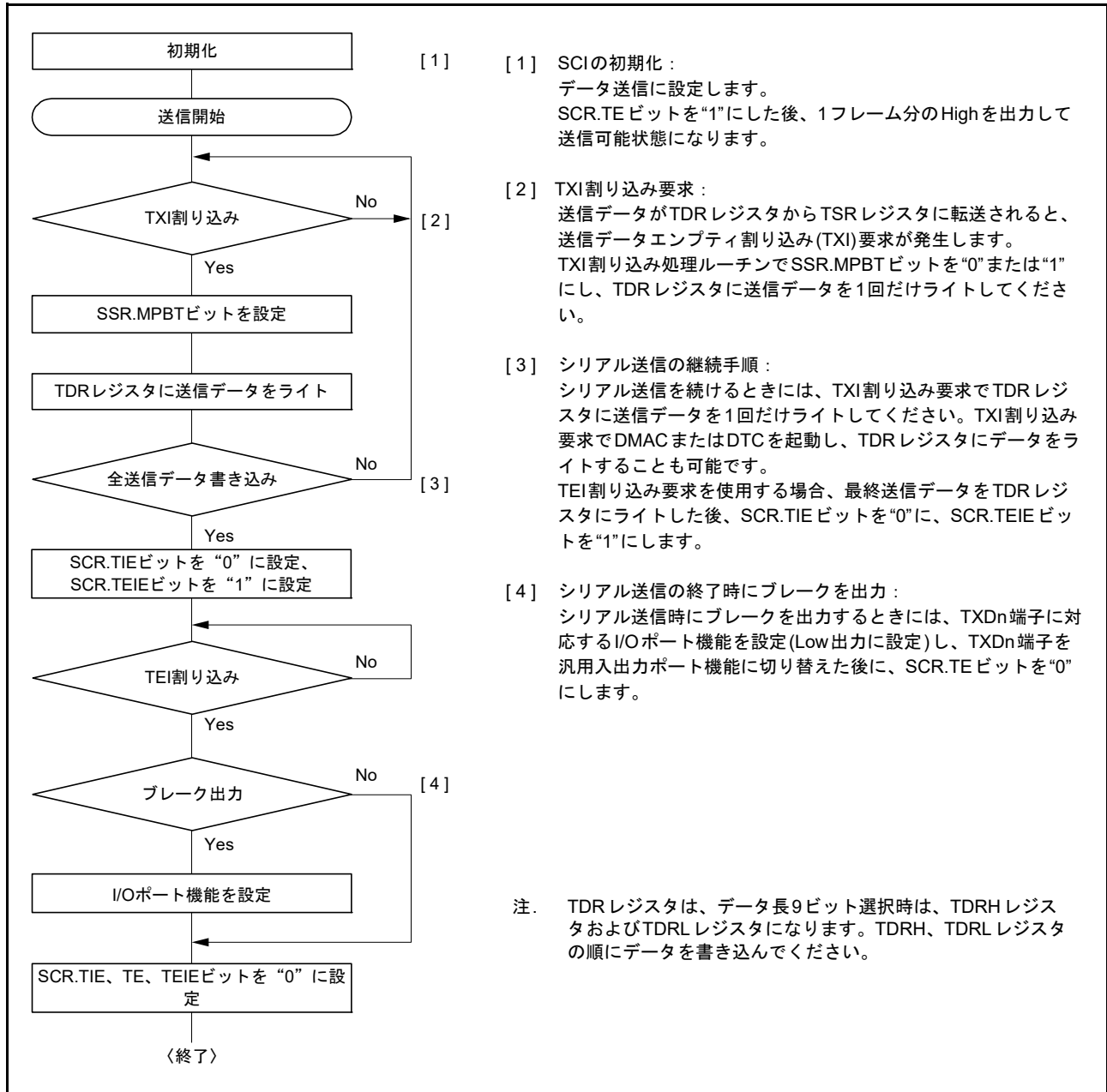
図 29.19 マルチプロセッサシリアル送信のフローチャートの例
