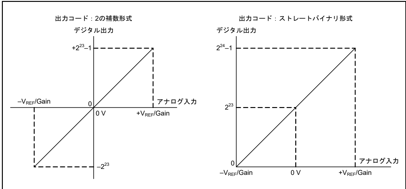
図 36.5 DSAD への入力電圧と A/D 変換結果
