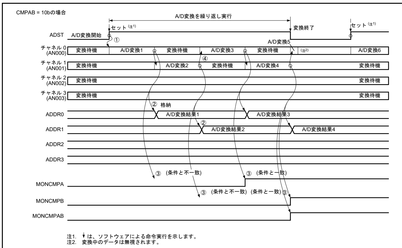
図 37.19 ウィンドウコンペア機能の動作例 (AN000、AN001、AN002、AN003 コンペア対象)
