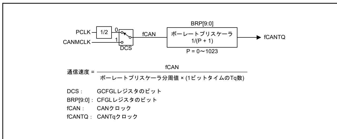
図 31.18 CAN クロック制御ブロック図
