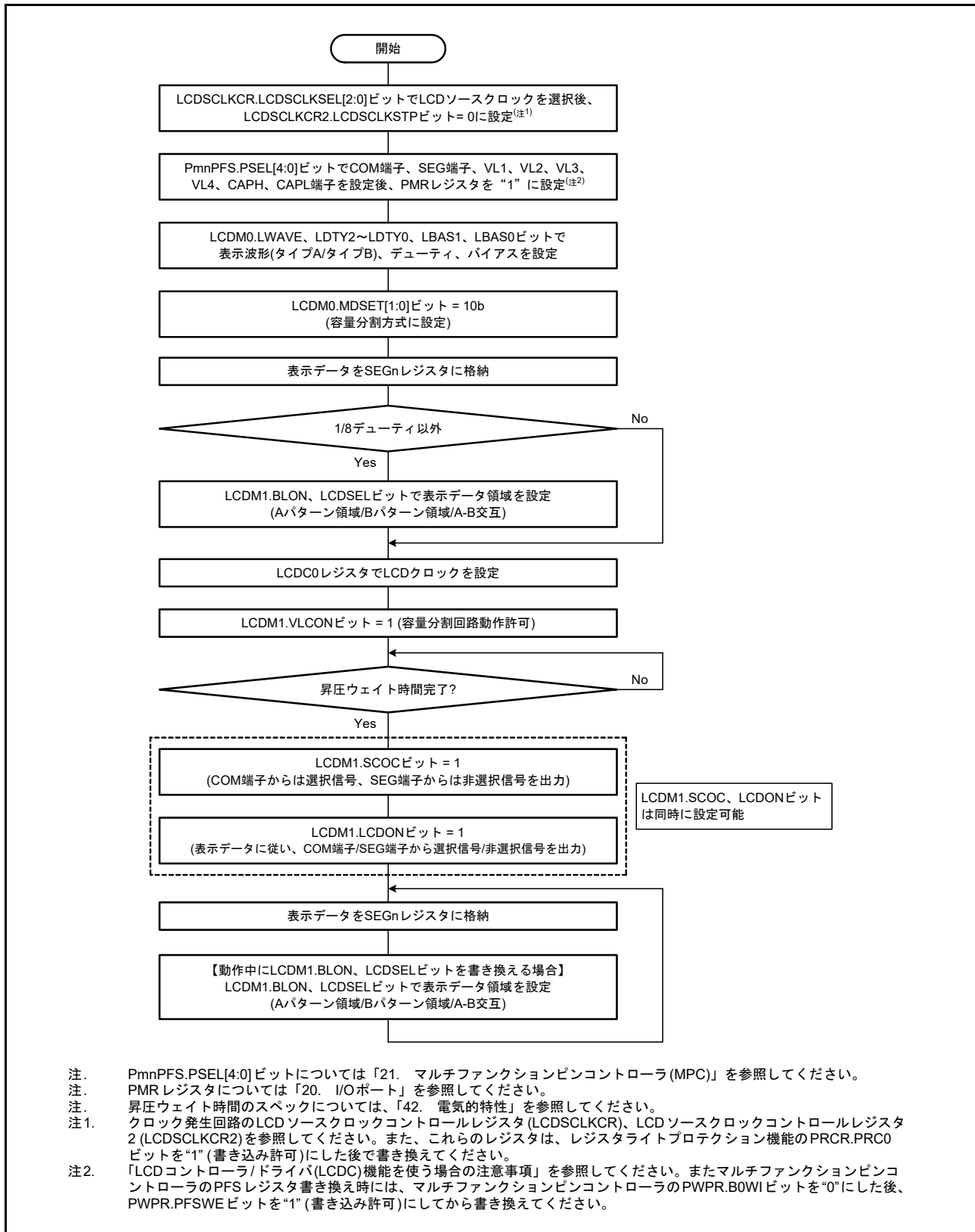
図 34.7 容量分割方式の設定手順
