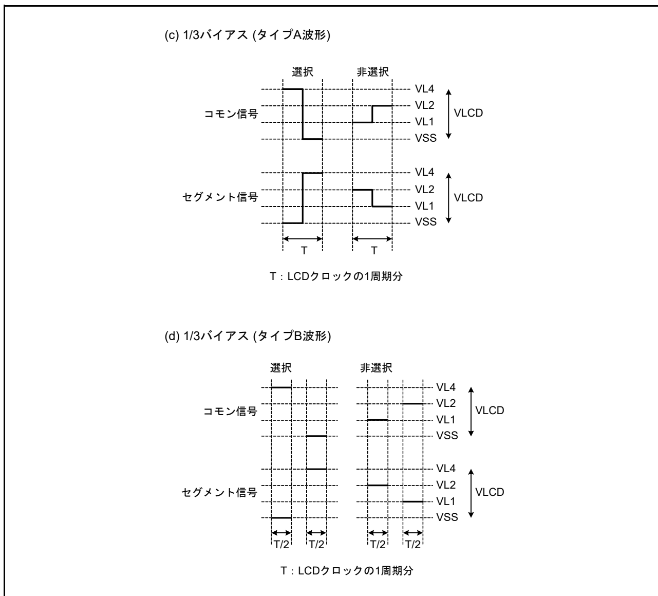
図 34.16 コモン信号とセグメント信号の電圧と位相 (2)
