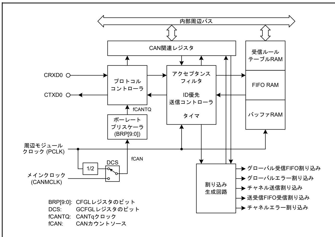
図 31.1 CANモジュールのブロック図
