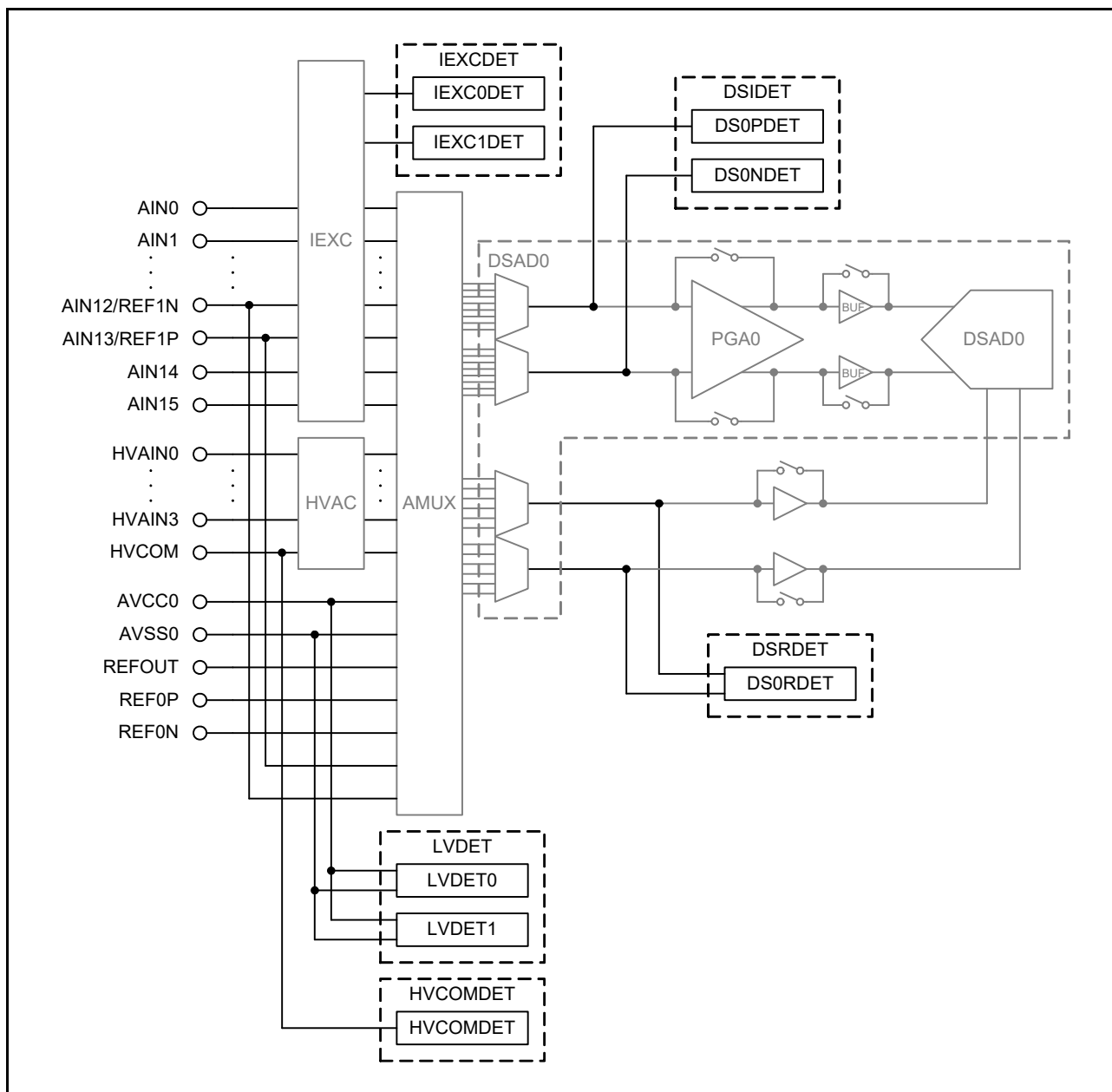
図 35.4 VDET のブロック図
