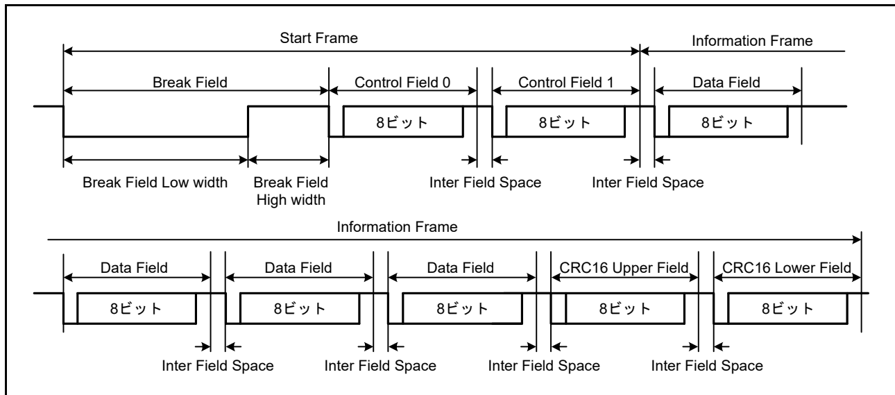
図 29.60 拡張シリアルモード制御部シリアル通信プロトコル
