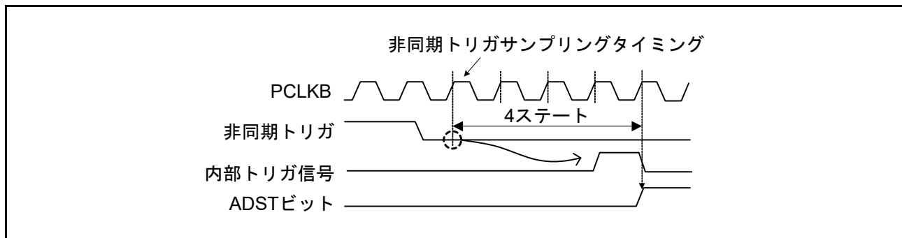
図 37.26 非同期トリガ入力タイミング
