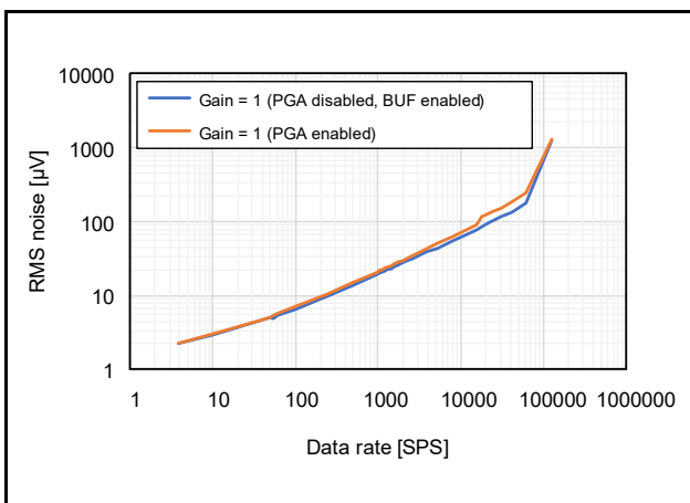
図 42.78 RMS ノイズのデータレート依存性 (AVCC0 = 5.0V、 T_a = 25^\circ\text{C} 、 f_{\text{MOD}} = 4\text{MHz} 、Sinc 4 フィルタまたは Sinc 4 +Sinc 4 フィルタ、 V_{\text{ID}} = 0\text{V} 、 V_{\text{REF}} = 2.5\text{V} 、リファレンスバッファ無効)
