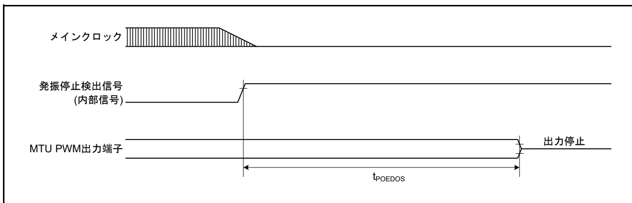
図 42.38 POE 出力ディセーブル時間 (発振停止検出)
