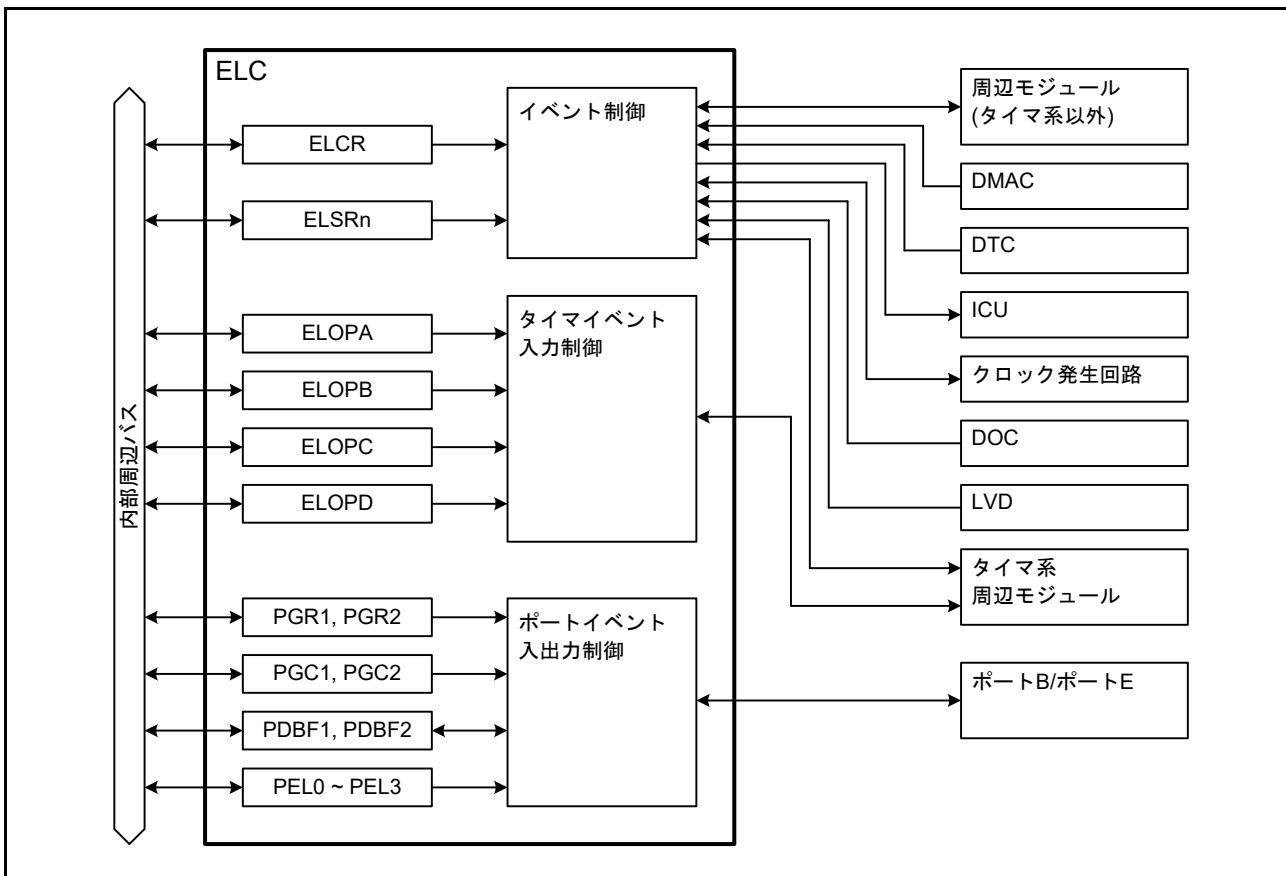
図 19.1 ELC のブロック図 (n = 1 ~ 4, 7, 8, 10, 12, 15, 16, 18 ~ 29, 46)
