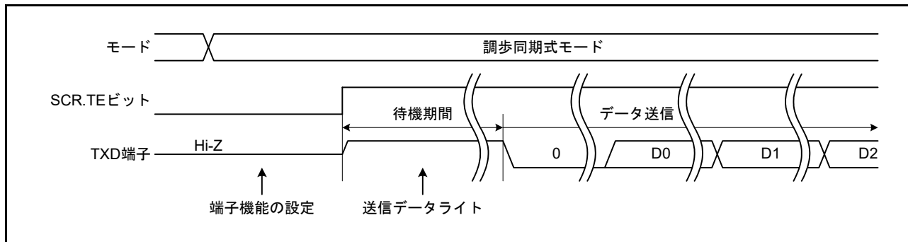
図 29.9 調歩同期式モード時のデータ送信タイミング例
