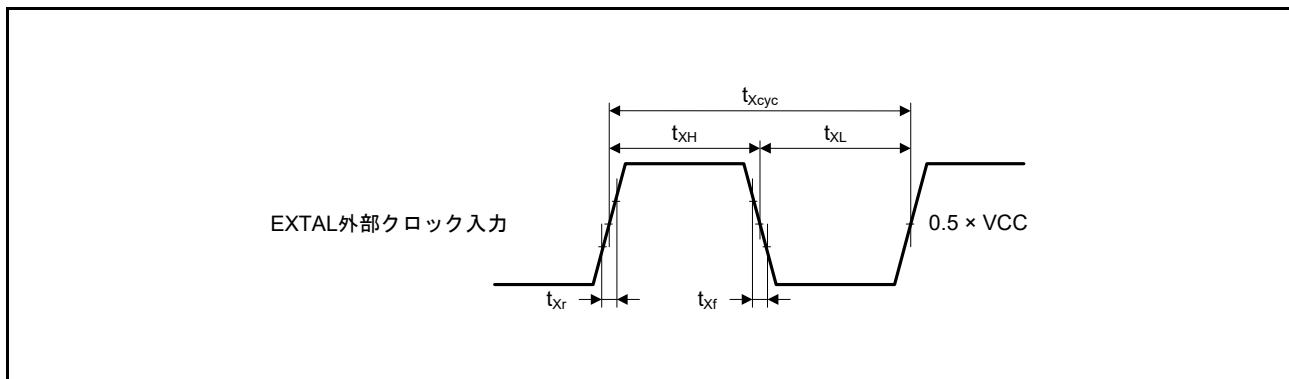
図 42.16 EXTAL 外部クロック入力タイミング
