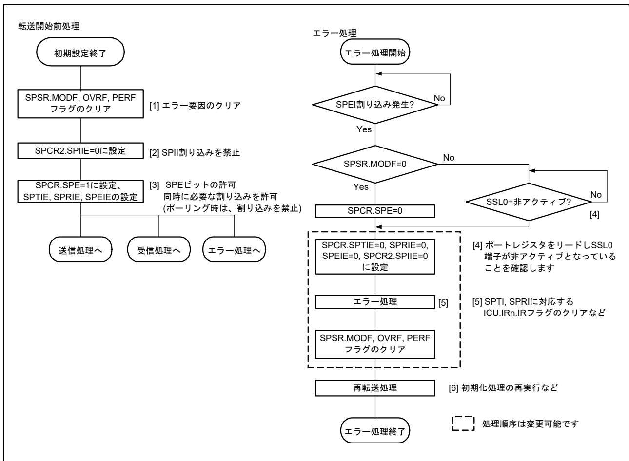
図 32.40 マスタモード時のフローチャート (エラー)
