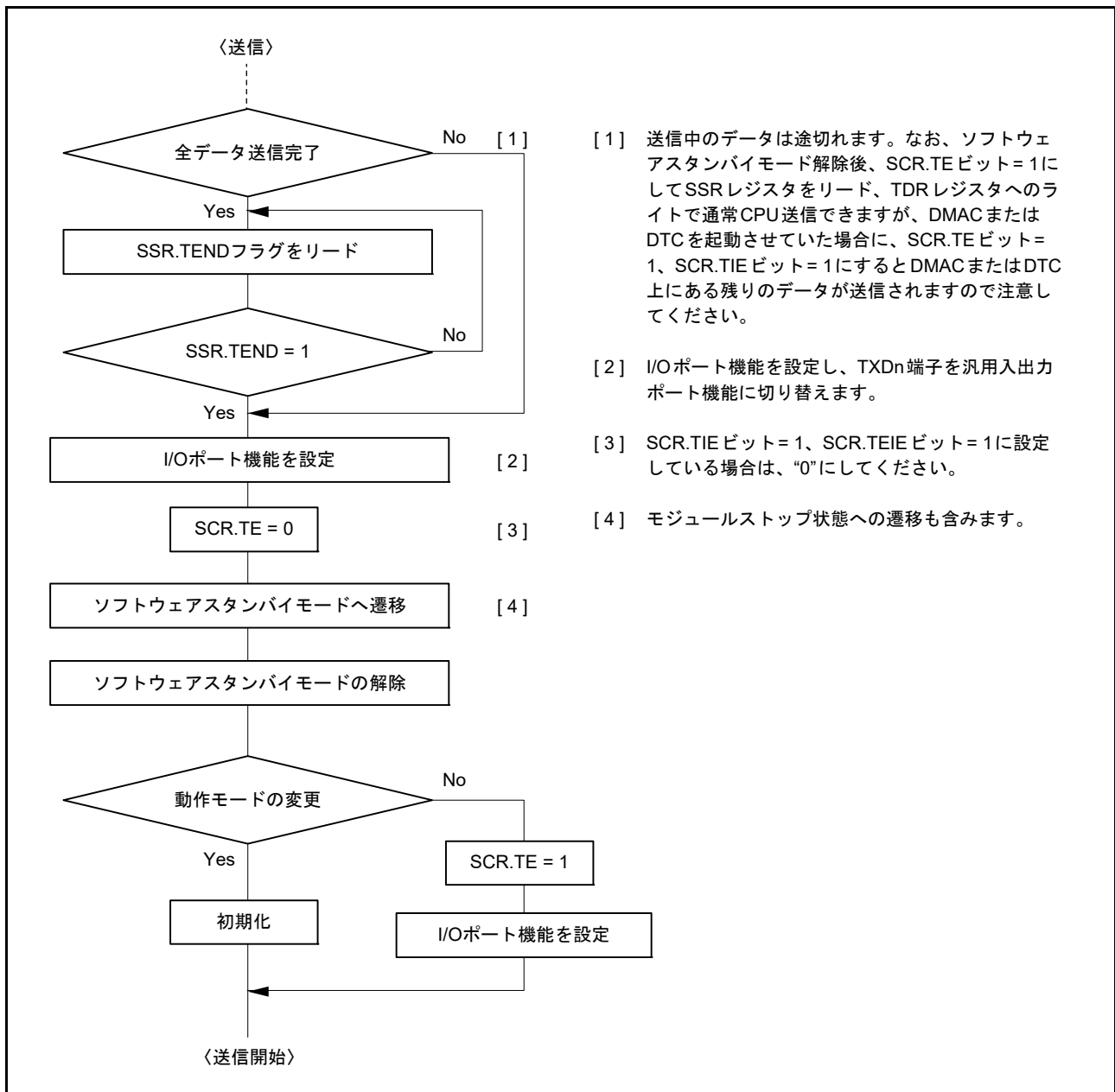
図 29.77 送信時のソフトウェアスタンバイモード遷移フローチャートの例
