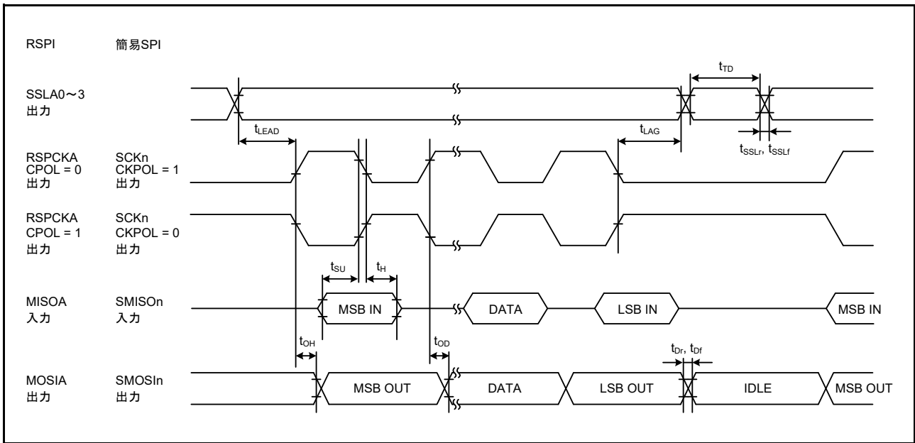
図 42.45 RSPCI タイミング (マスタ、CPHA = 1)/ 簡易 SPI クロックタイミング (マスタ、CKPH = 0) (n = 0, 1, 5, 6, 8, 9, 12)
