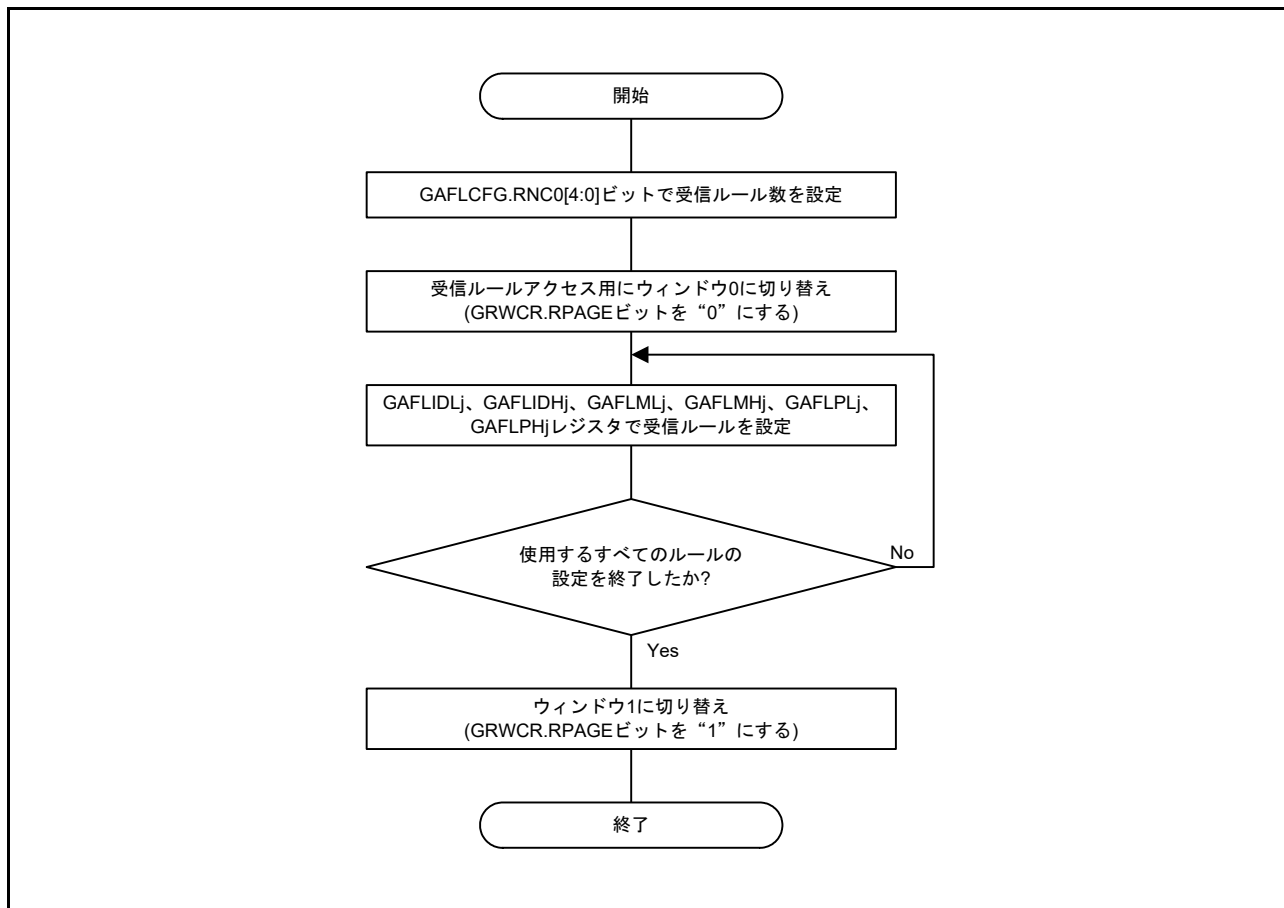
図 31.19 受信ルール設定手順
