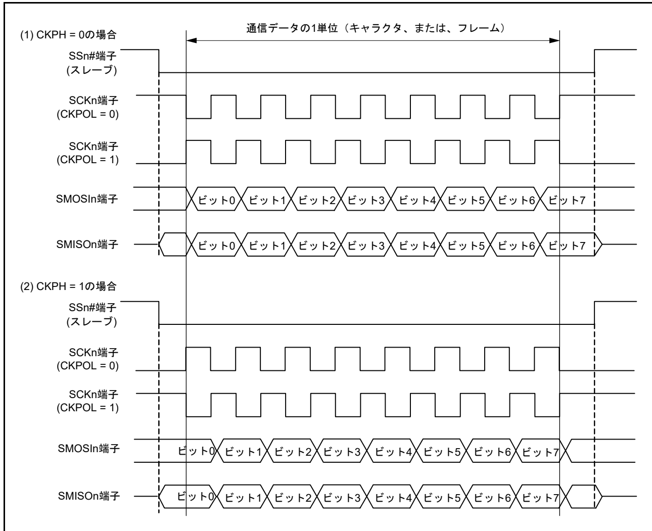
図 29.58 簡易 SPI モードのクロックと送受信データの関係
