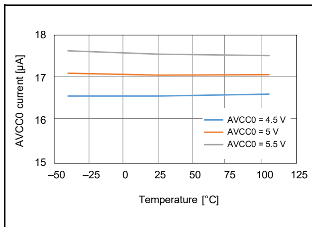
図 42.8 24 ビット \Delta - \Sigma A/D コンバータ動作電流の温度依存性 (PGA 有効)
