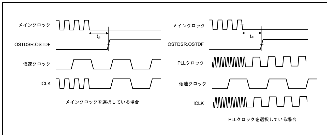
図 42.56 発振停止検出タイミング
