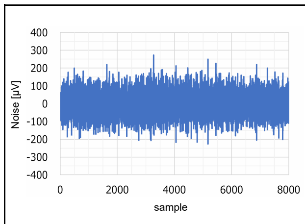
図 42.58 ノイズプロット (AVCC0 = 5.0V、 T_a = 25^\circ\text{C} 、Gain = 1 (PGA 無効、BUF 無効)、 f_{\text{MOD}} = 4\text{MHz} 、 f_{\text{DR}} = 125\text{k SPS} 、Sinc 5 フィルタ、 V_{\text{ID}} = 0\text{V} 、 V_{\text{REF}} = 2.5\text{V} 、リファレンスバッファ無効)
