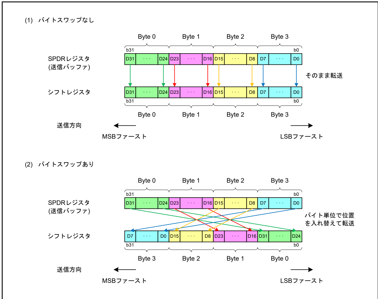
図 32.22 MSB/LSB ファーストとバイトスワップあり / なしの設定と送信データ変換
