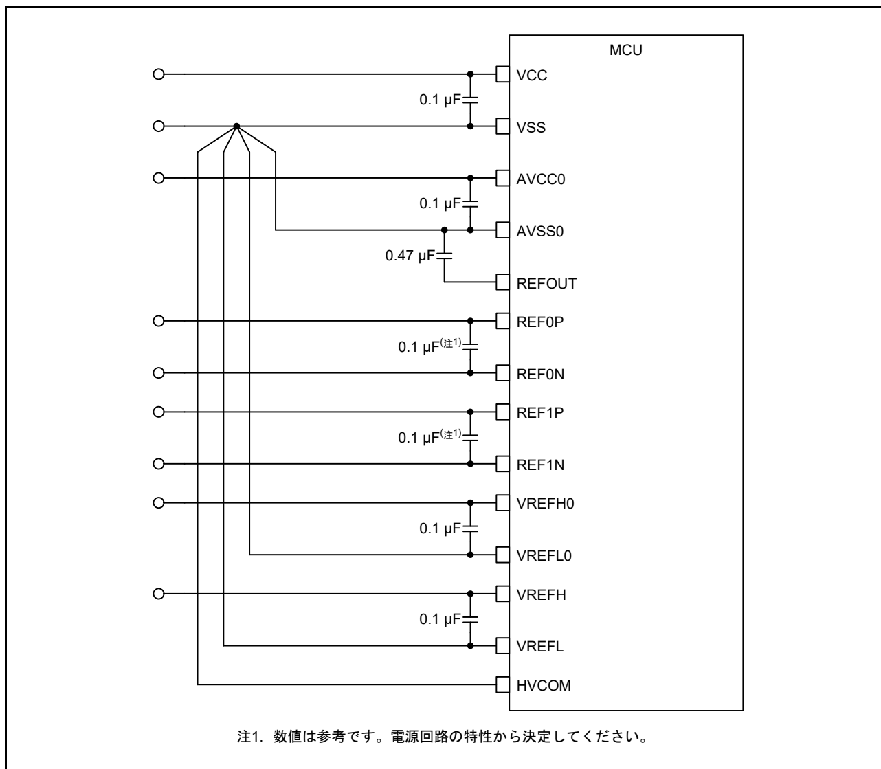
図 35.17 電源端子、基準電圧入力端子の接続例
