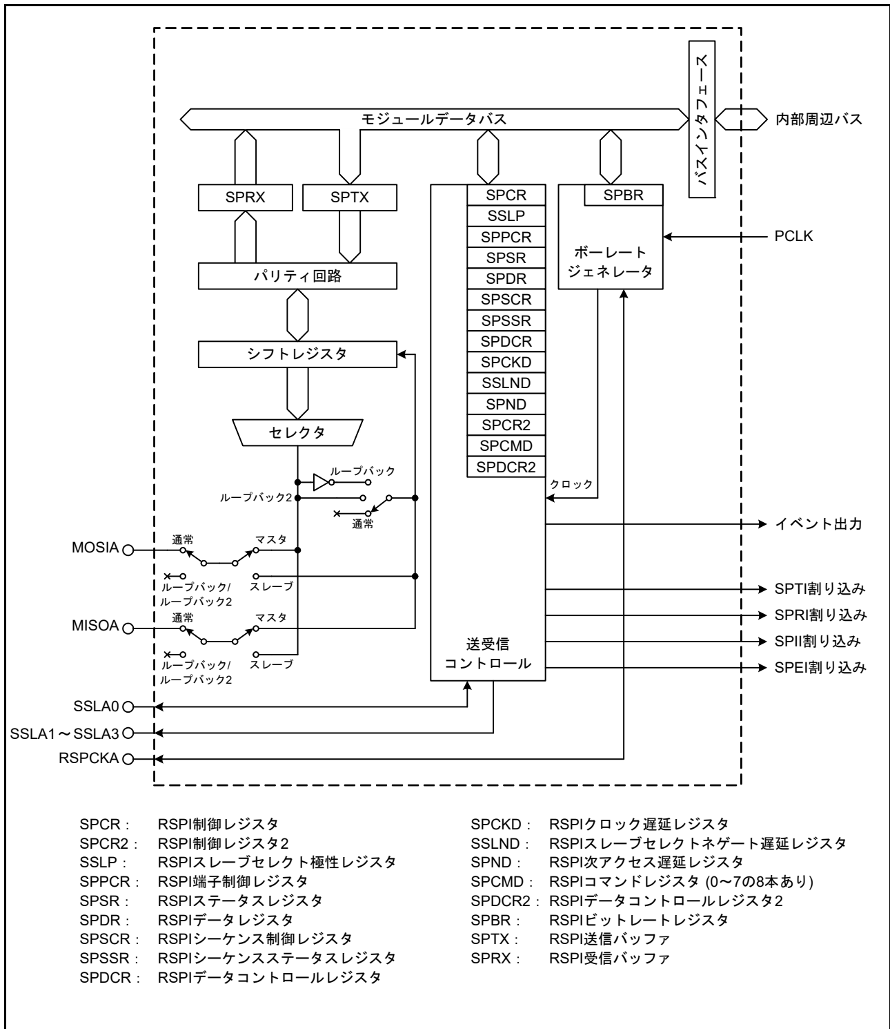
図 32.1 RSPI のブロック図
