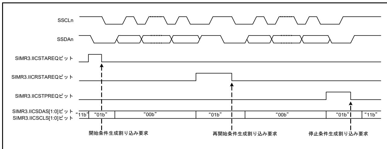
図 29.48 開始条件、再開条件、停止条件生成の動作タイミング
