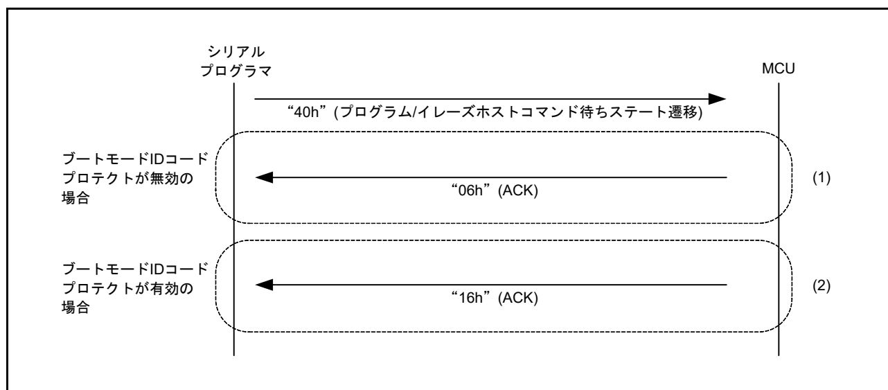
図 41.33 プログラム/イレーズホストコマンド待ち状態への遷移手順
