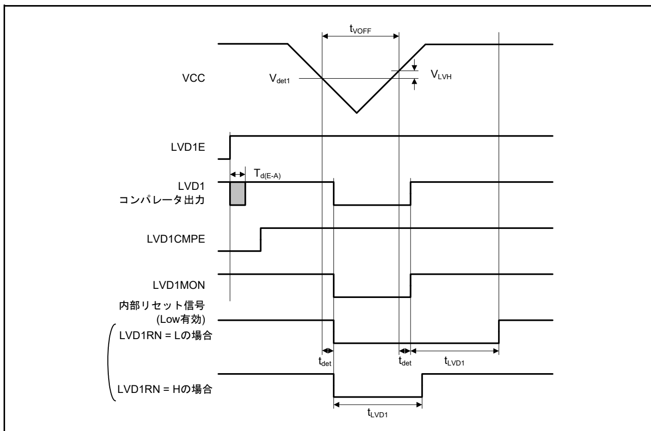
図 42.54 電圧検出回路タイミング (V det1 )
