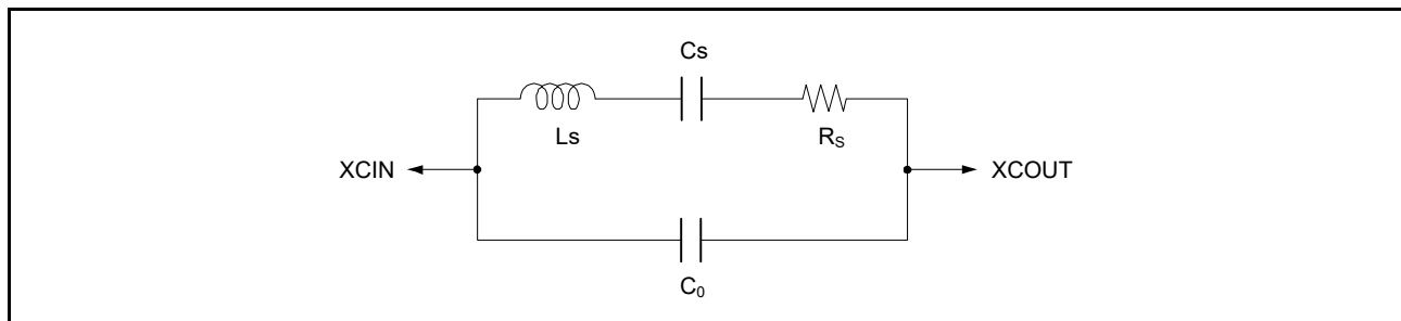
図 9.6 水晶振動子の等価回路
