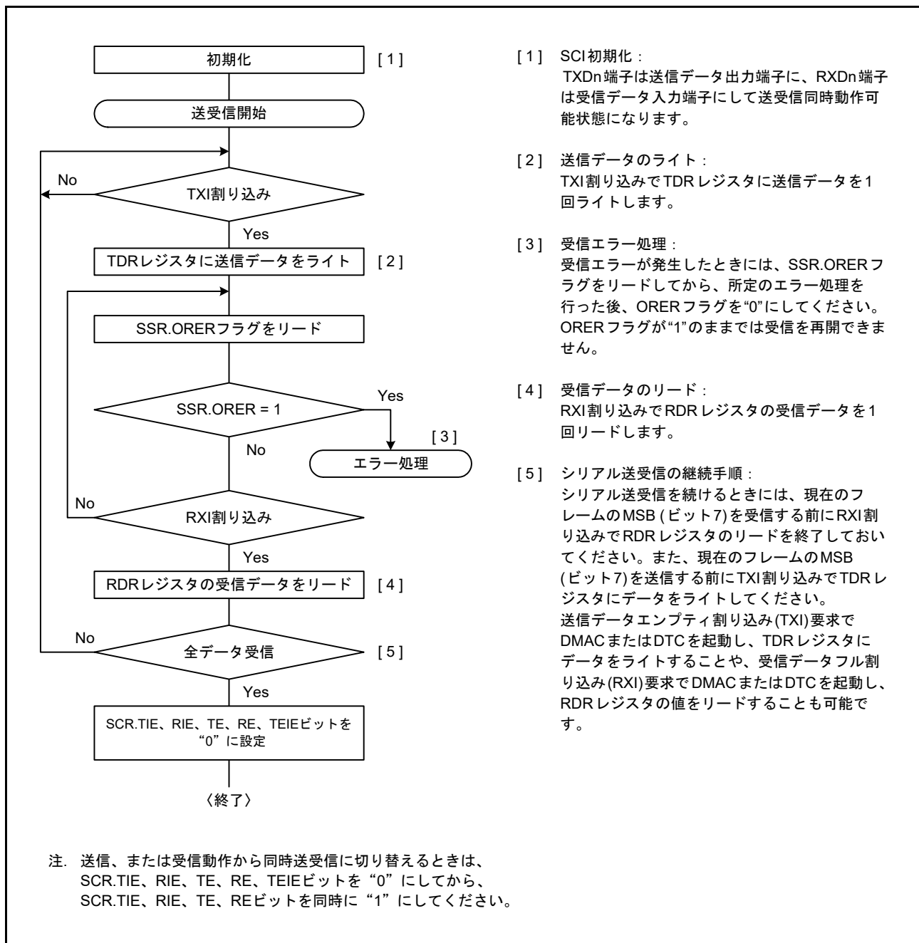
図 29.32 クロック同期式モードのシリアル送受信同時動作のフローチャート例
