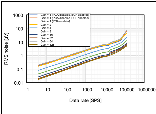
図 42.65 RMS ノイズのデータレート依存性 (AVCC0 = 5.0V、 T_a = 25^\circ\text{C} 、 f_{\text{MOD}} = 4\text{MHz} 、Sinc 5 フィルタまたは Sinc 5 +Sinc 1 フィルタ、 V_{\text{ID}} = 0\text{V} 、 V_{\text{REF}} = 2.5\text{V} 、リファレンスバッファ無効)
