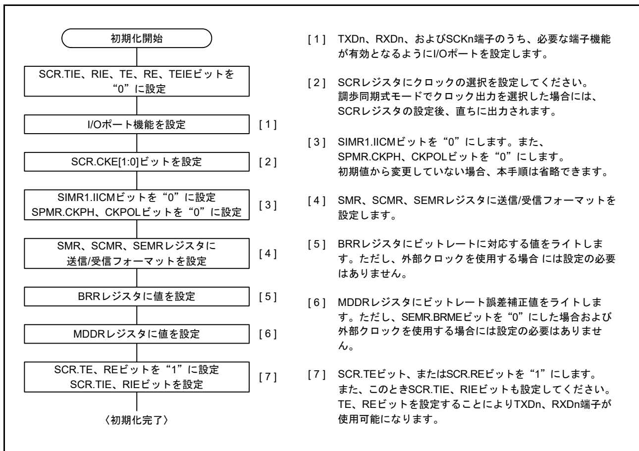
図 29.8 SCIの初期化フローチャートの例 (調歩同期式モード)
