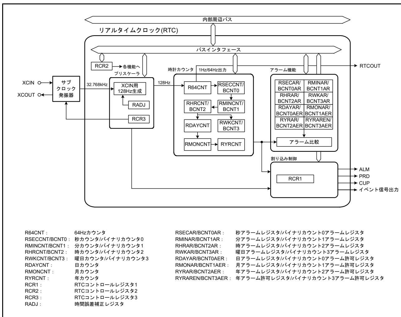
図 26.1 RTCのブロック図
