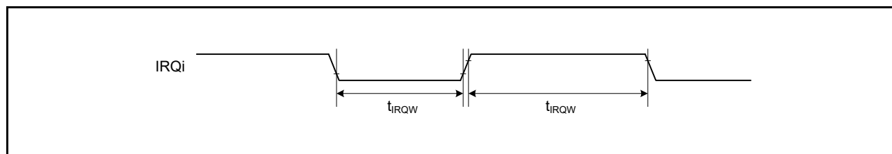
図 42.30 IRQ 割り込み入力タイミング
