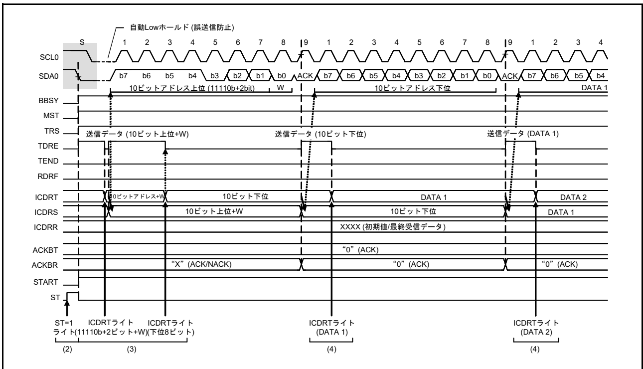
図 30.7 マスタ送信の動作タイミング (2) (10ビットアドレスフォーマットのとき)
