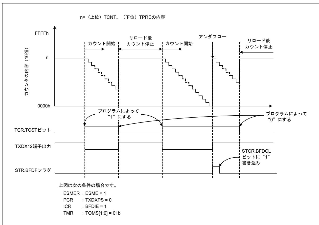
図 29.73 Break Field Low width 出力モードの動作例
