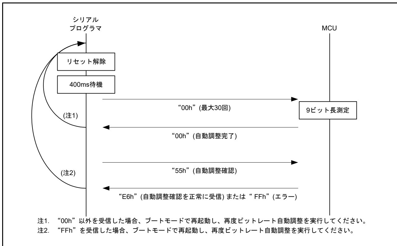
図 41.30 ビットレート自動調整の手順
