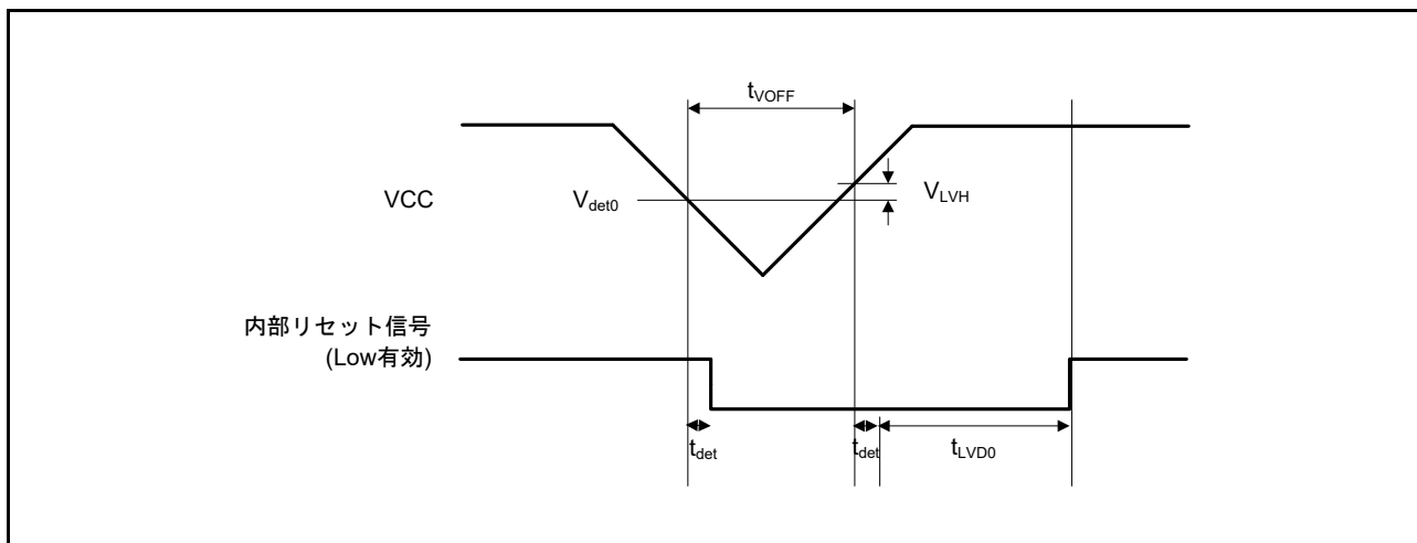
図 42.53 電圧検出回路タイミング (Vdet0)
