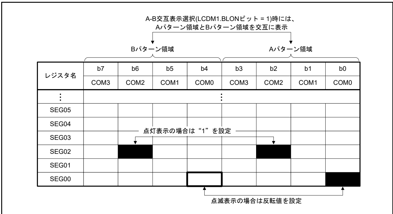
図 34.2 A-B 交互表示モード時の LCD 表示データレジスタの設定例
