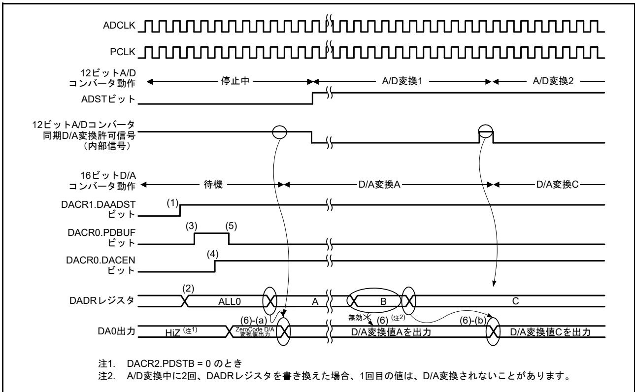
図 38.3 16ビットD/Aコンバータを12ビットA/Dコンバータに同期して変換する例
