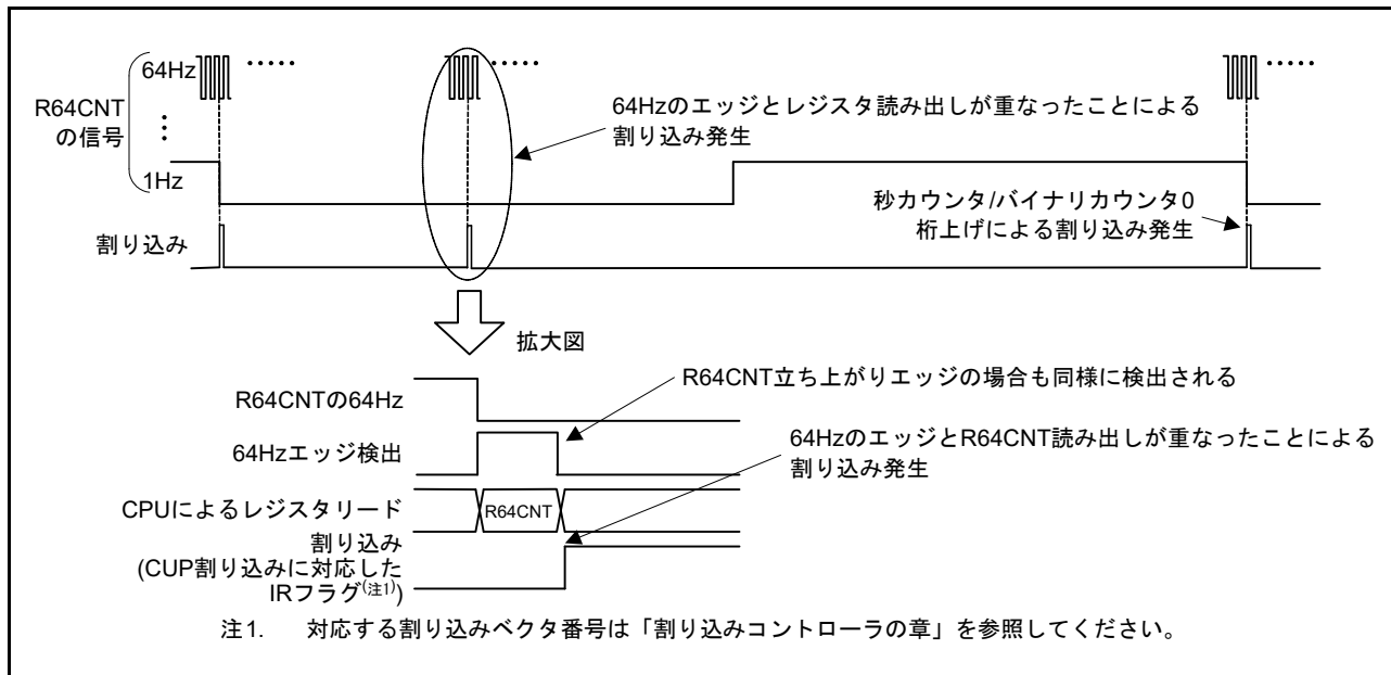
図 26.10 桁上げ割り込み (CUP) のタイミングチャート
