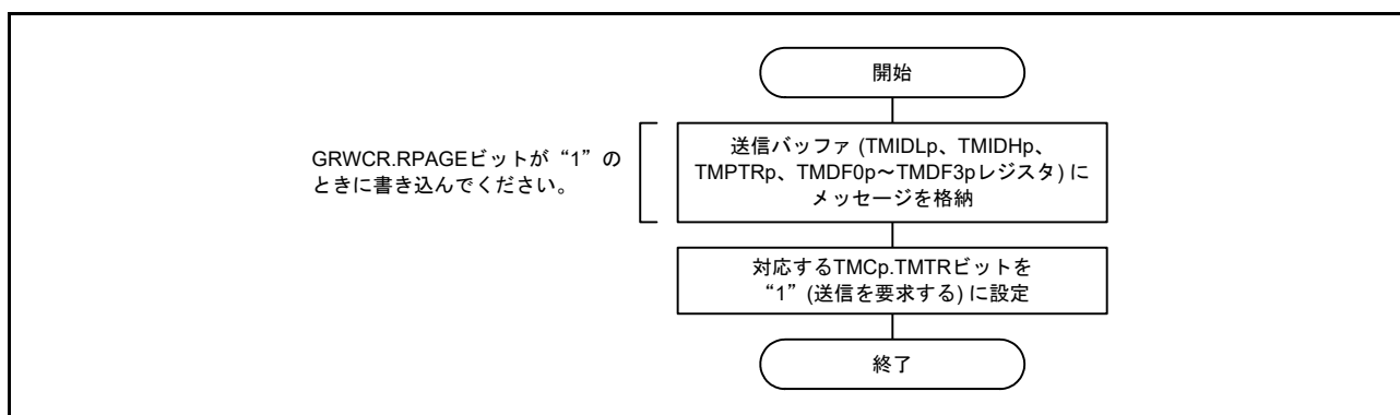
図 31.26 送信バッファからの送信手順
