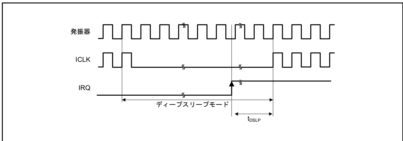
図 42.28 ディープスリープモード解除タイミング
