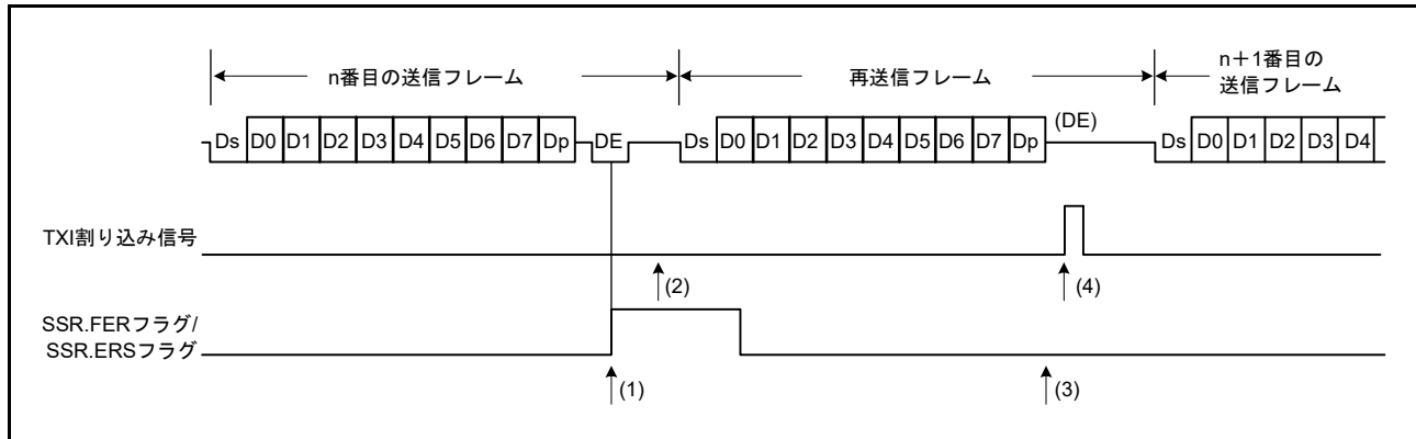
図 29.40 SCI 送信モードの場合の再送信動作 (送信時の再送信動作)
