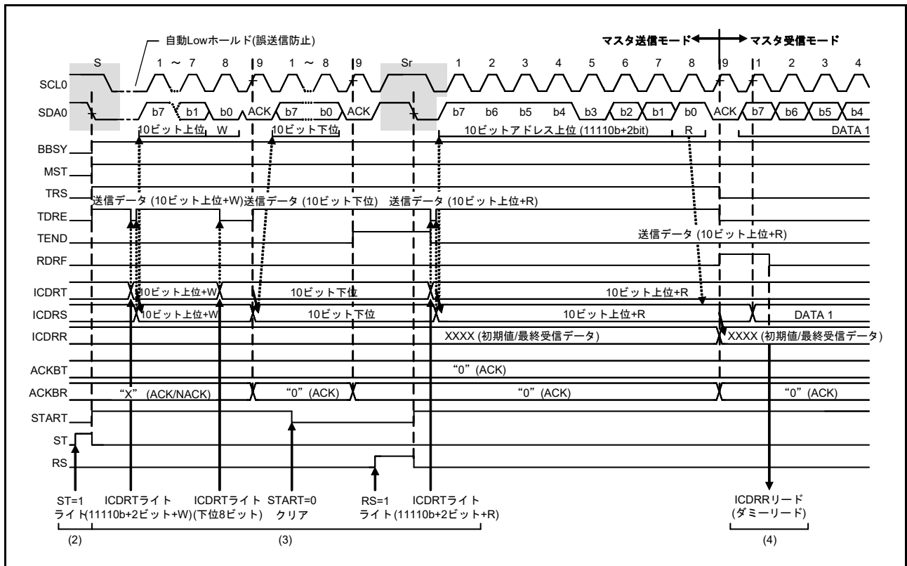
図 30.12 マスタ受信の動作タイミング (2) (10 ビットアドレスフォーマット、RDRFS ビット = 0 のとき)
