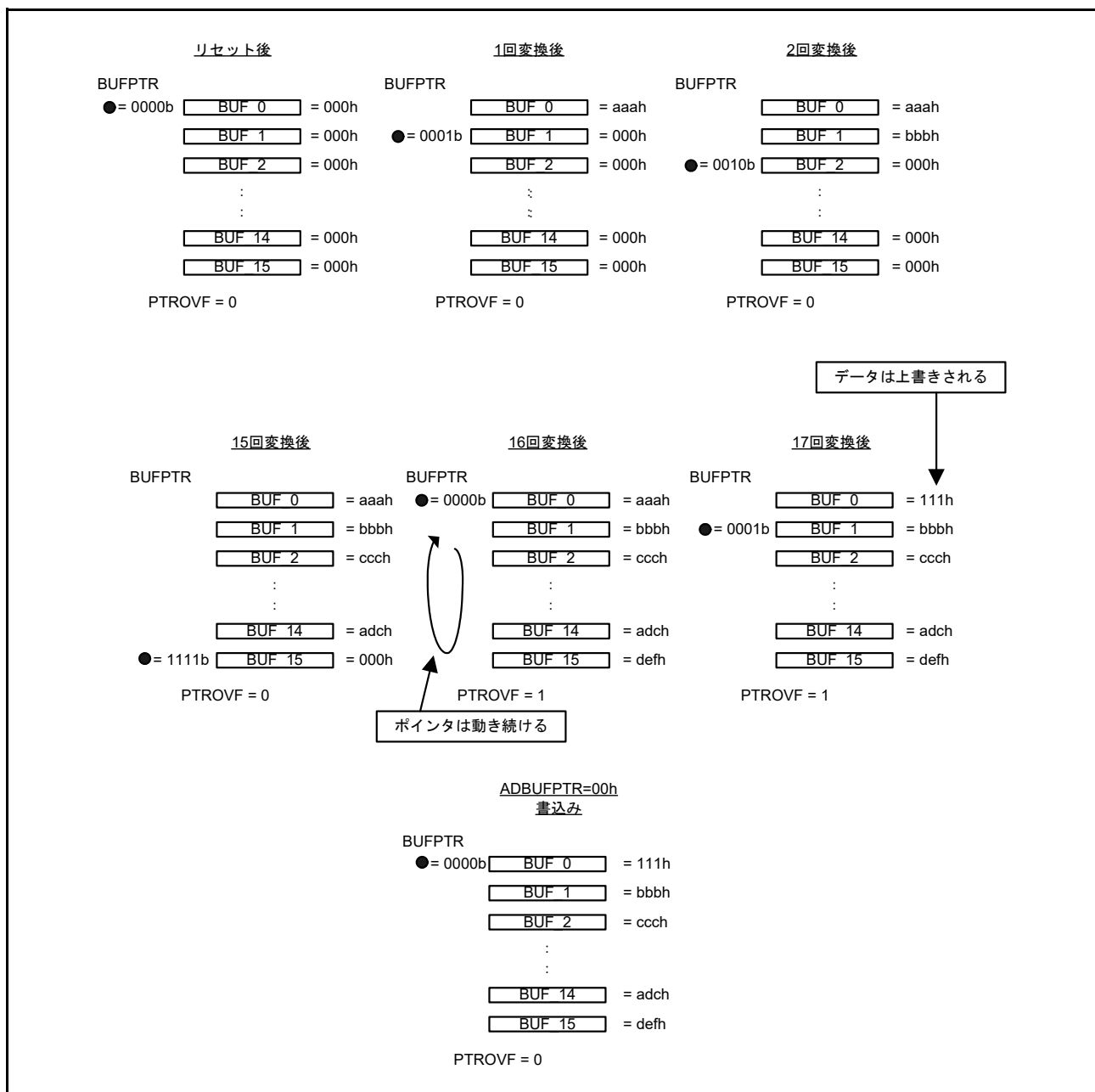
図 37.20 データ格納バッファとポインタ、オーバフローフラグの動作概要
