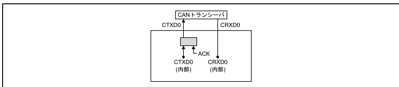
図 31.11 セルフテストモード 0 選択時の接続
