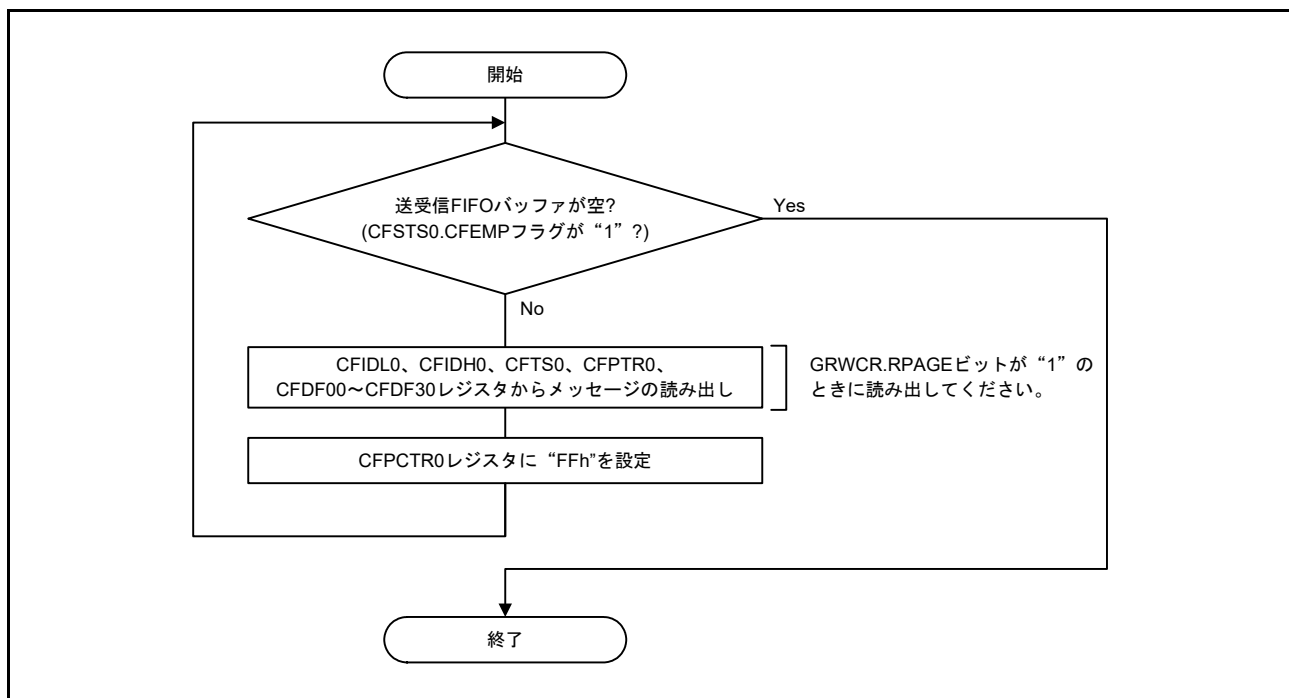
図 31.24 送受信 FIFO バッファの読み出し手順
