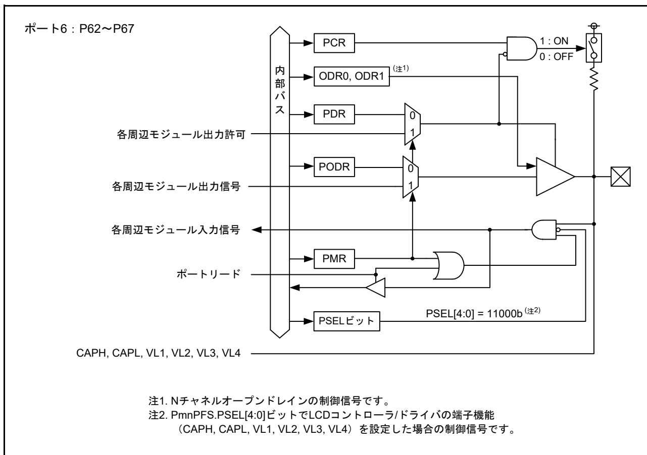
図 20.4 入出力ポートの構成 (4)
