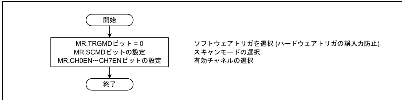
図 36.17 チャネル共通設定フロー
