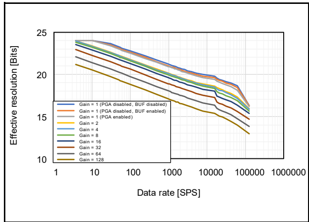
図 42.66 有効分解能のデータレート依存性 (AVCC0 = 5.0V、 T_a = 25^\circ\text{C} 、 f_{\text{MOD}} = 4\text{MHz} 、Sinc 5 フィルタまたは Sinc 5 +Sinc 1 フィルタ、 V_{\text{ID}} = 0\text{V} 、 V_{\text{REF}} = 2.5\text{V} 、リファレンスバッファ無効)
