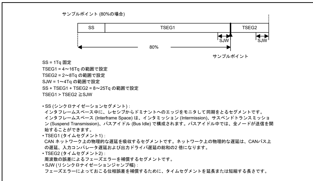
図 31.17 ビットタイミング図
