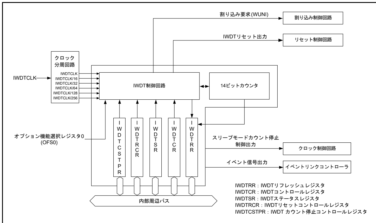
図 28.1 IWDT のブロック図
