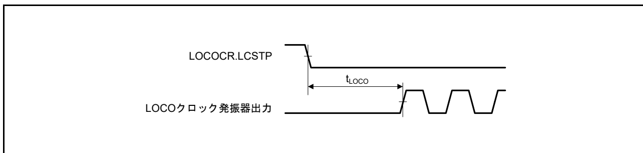
図 42.18 LOCO クロック発振開始タイミング
