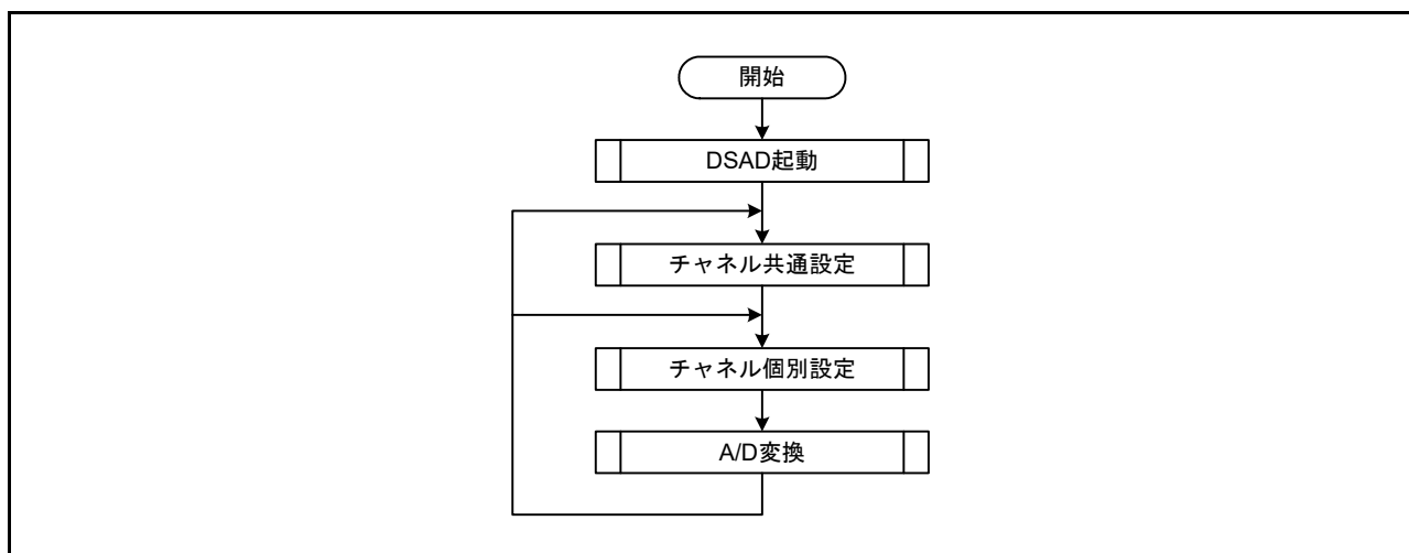
図 36.15 全体フロー
