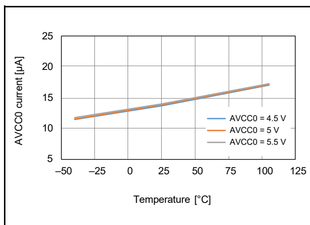
図 42.10 温度センサ動作電流の温度依存性
