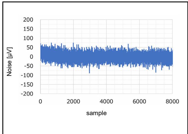
図 42.77 ノイズプロット (AVCC0 = 5.0V、 T_a = 25^\circ\text{C} 、Gain = 1 (PGA 有効、BUF 有効)、 f_{\text{MOD}} = 4\text{MHz} 、 f_{\text{DR}} = 976.6\text{ SPS} 、Sinc 4 +Sinc 4 フィルタ、 V_{\text{ID}} = 0\text{V} 、 V_{\text{REF}} = 2.5\text{V} )
