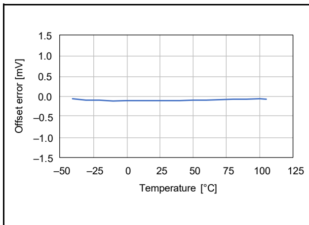
図 42.99 オフセットエラーの温度依存性 (AVCC0 = 5V, VREFH = 5V)
