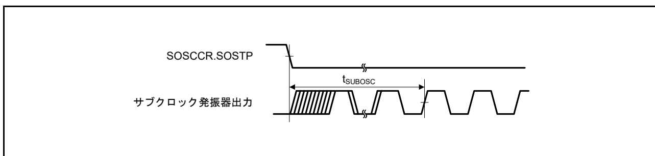
図 42.23 サブクロック発振開始タイミング
