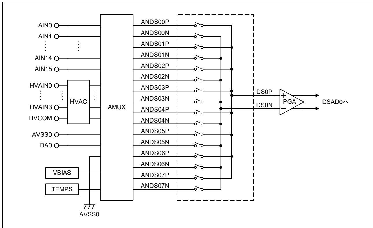
図 36.2 アナログ入力チャンネルのブロック図
