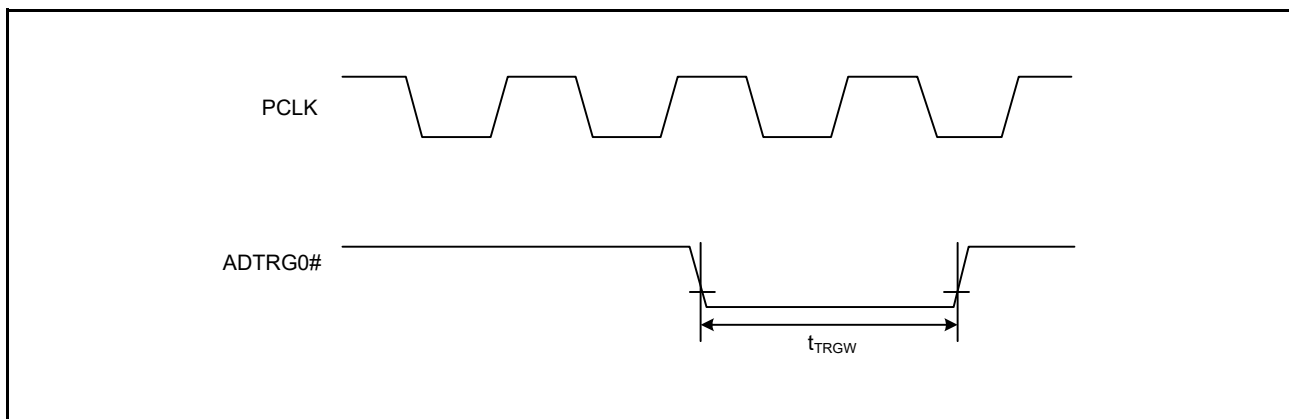
図 42.48 A/D コンバータ外部トリガ入力タイミング
