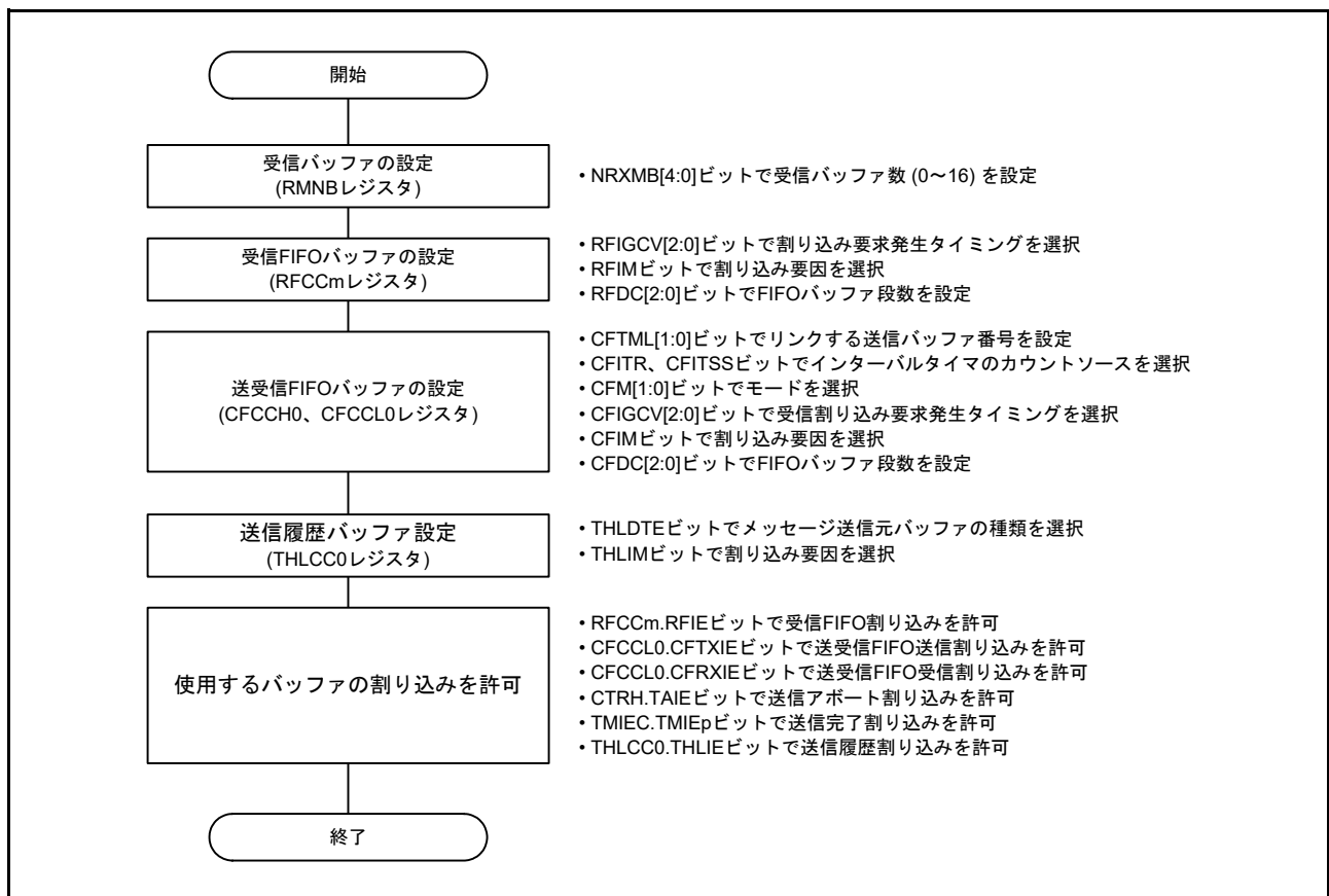
図 31.21 各種バッファの設定手順
