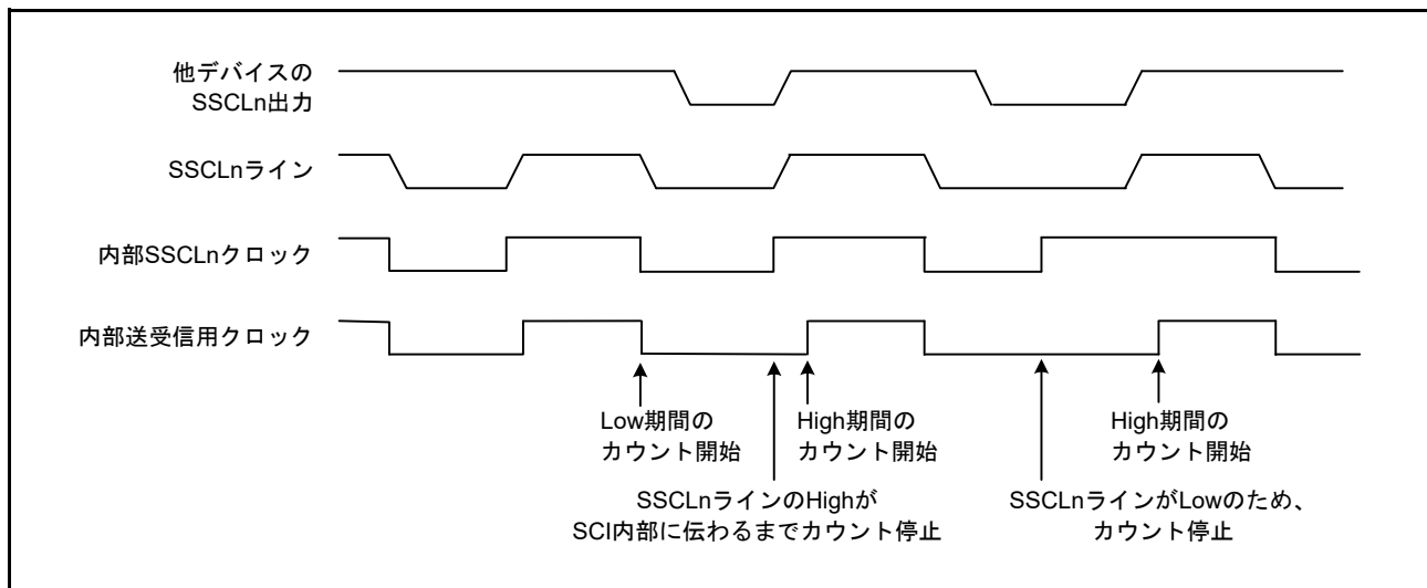
図 29.49 クロック同期化の動作例
