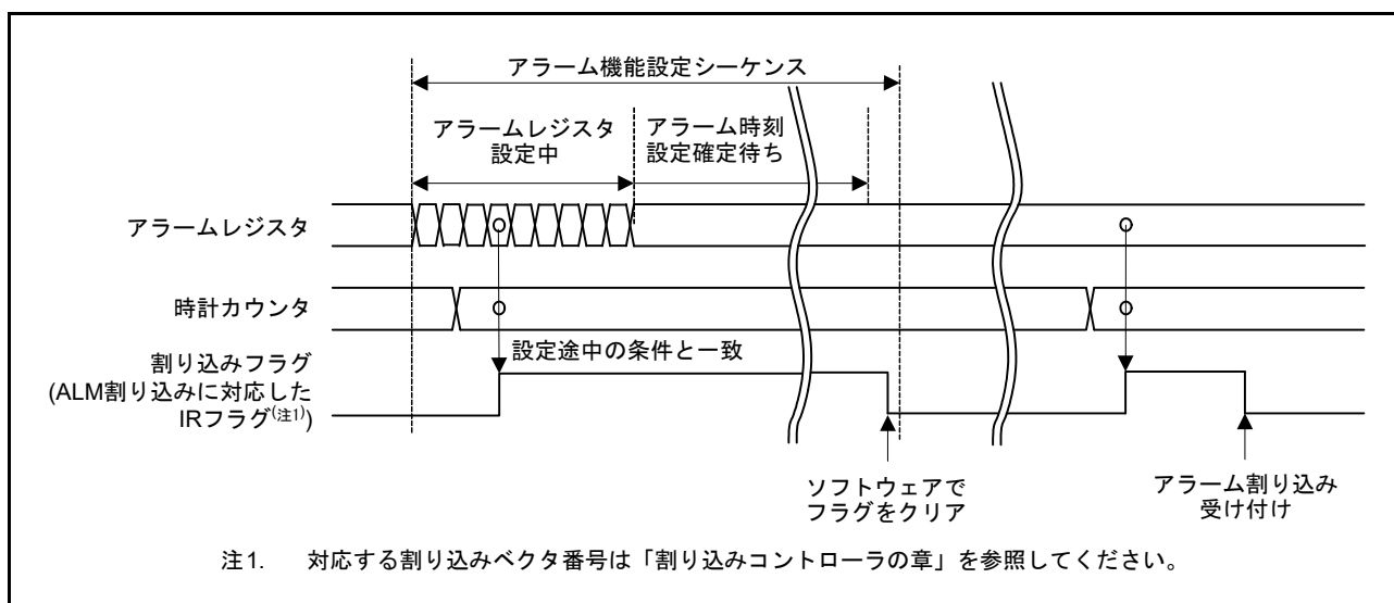
図 26.9 アラーム割り込み (ALM) のタイミングチャート
