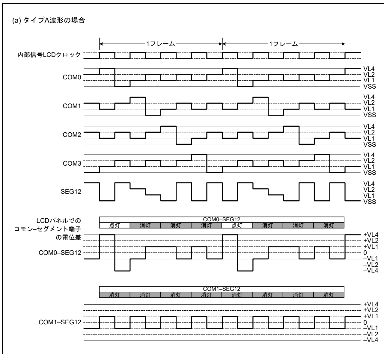
図 34.30 SEG12 端子と各コモン端子間の 1/4 デューティ LCD 駆動波形例 (1/3 バイアス) (1)
