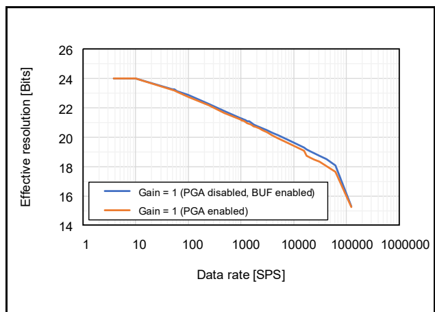
図 42.79 有効分解能のデータレート依存性 (AVCC0 = 5.0V、 T_a = 25^\circ\text{C} 、 f_{\text{MOD}} = 4\text{MHz} 、Sinc 4 フィルタまたは Sinc 4 +Sinc 4 フィルタ、 V_{\text{ID}} = 0\text{V} 、 V_{\text{REF}} = 2.5\text{V} 、リファレンスバッファ無効)
