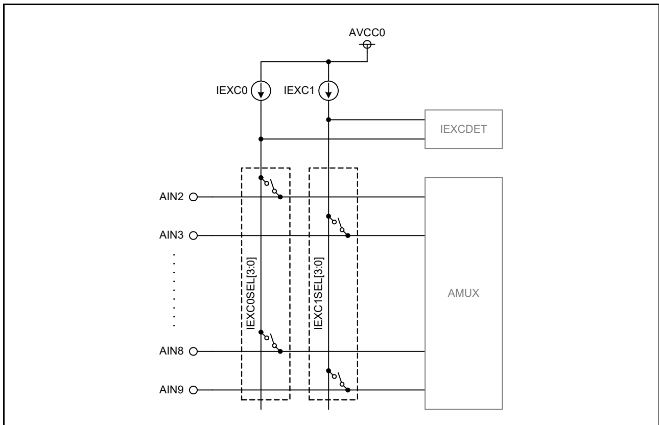
図 35.3 IEXC のブロック図
