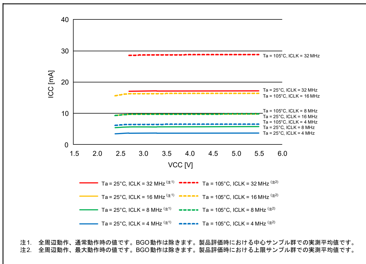
図 42.1 高速動作モードの電圧依存性 (参考データ)
