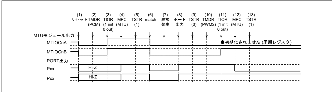
図 22.145 位相計数モードで異常が発生し、PWM モード2で復帰する場合
