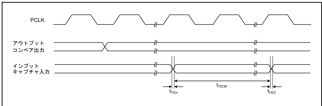
図 42.32 MTU入出力タイミング
