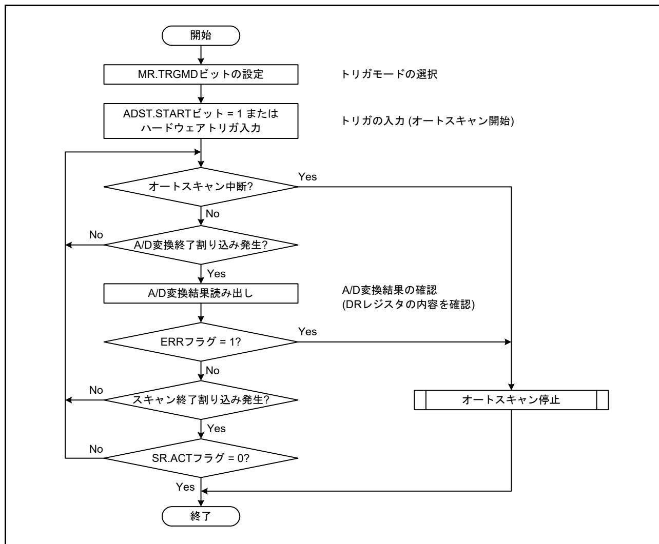
図 36.19 A/D 変換フロー
