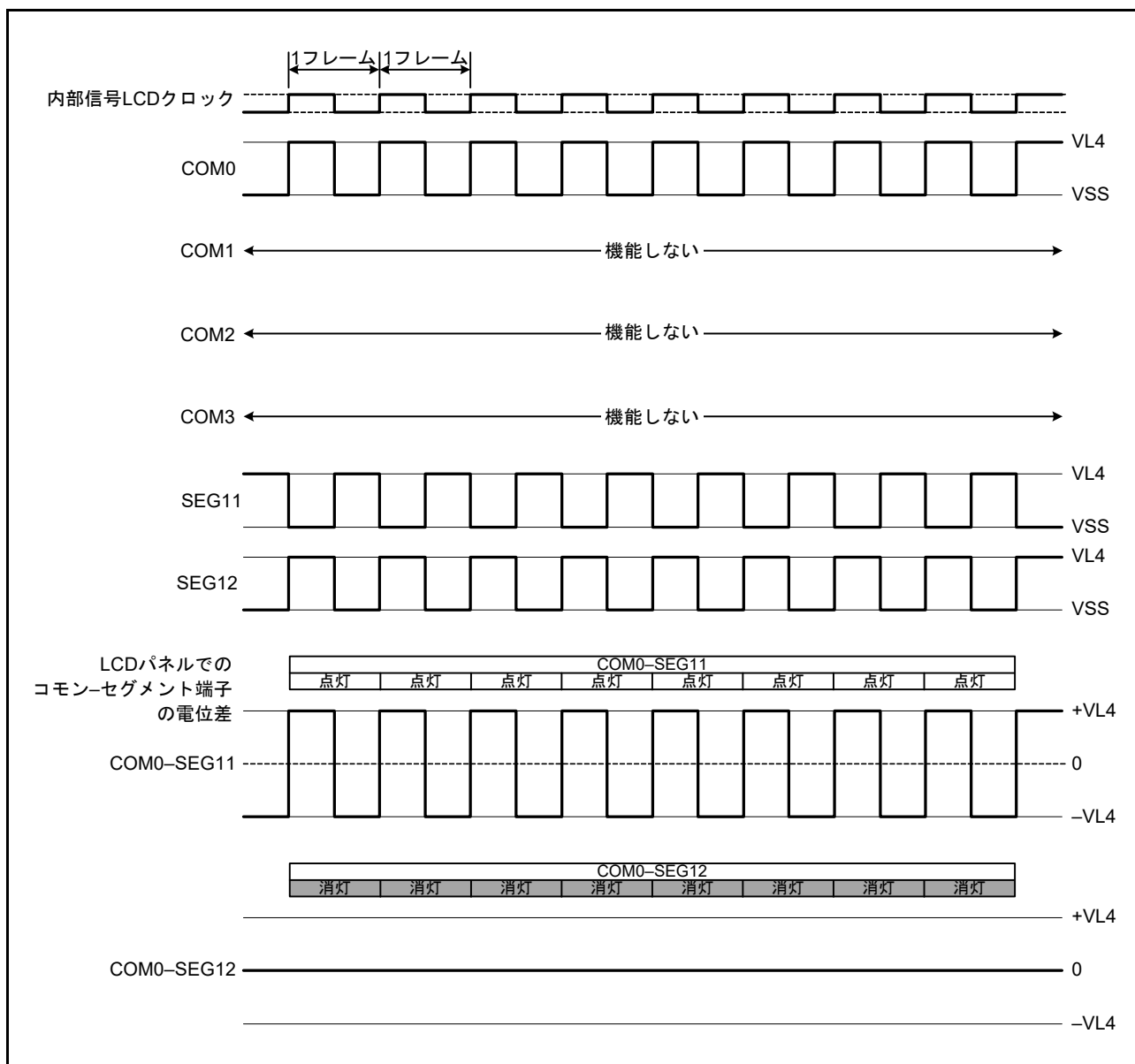
図 34.20 SEG11、SEG12 端子と COM0 端子間のスタティック LCD 駆動波形例
