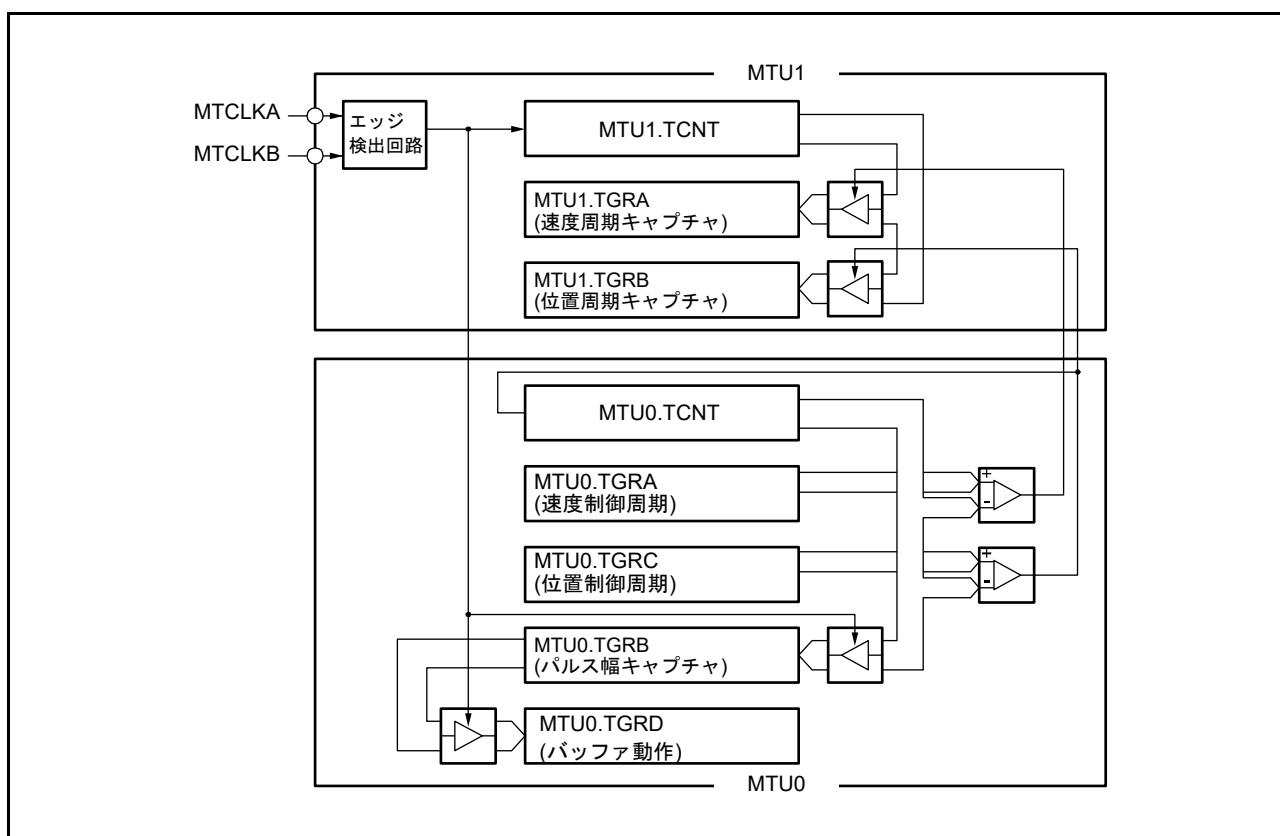
図 22.34 位相計数モードの応用例
