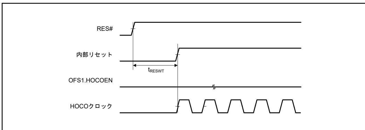
図 42.20 HOCO クロック発振開始タイミング (OFS1.HOCOEN ビット “0” 設定時のリセット解除後)
