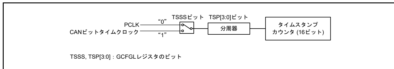
図 31.6 タイムスタンプ機能のブロック図
