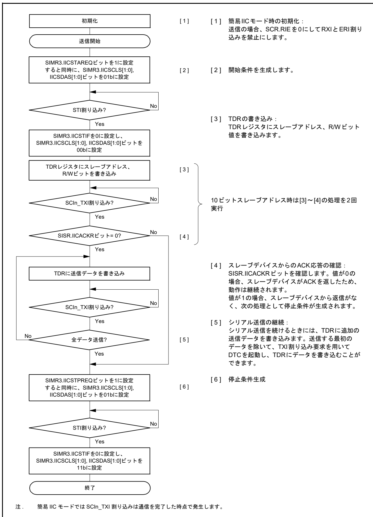
図 27.66 簡易 IIC モードのマスタ送信の手順例 (送信割り込み、受信割り込み使用時)
