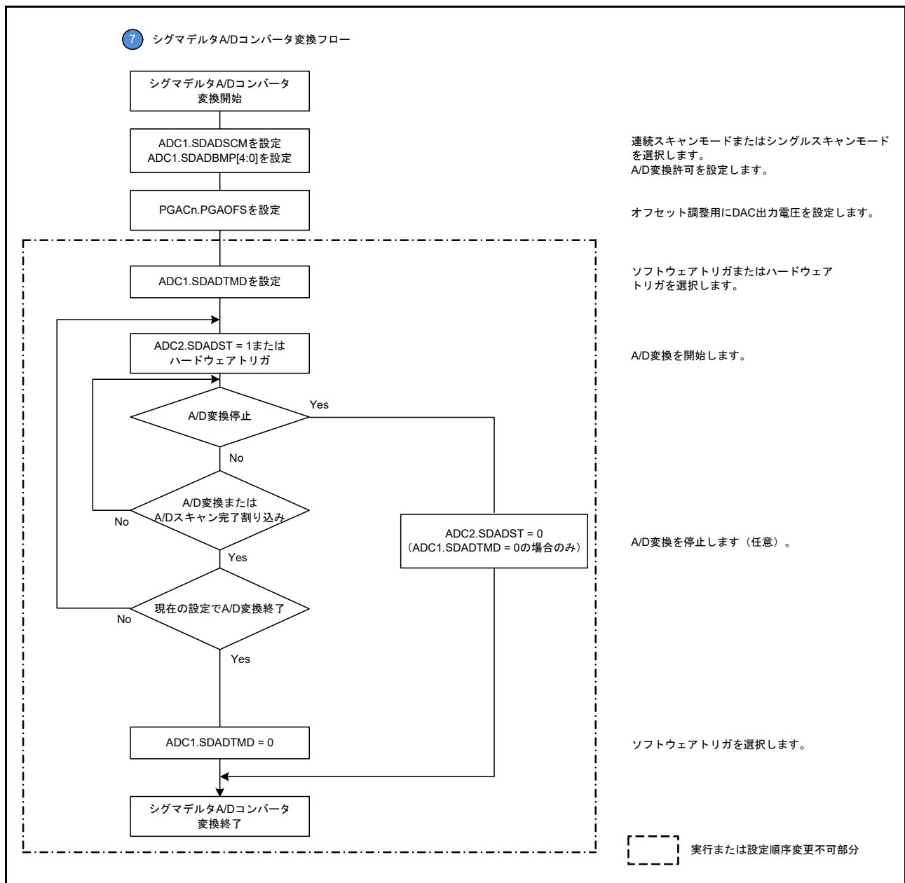
図 33.29 SDADC24 変換フロー
