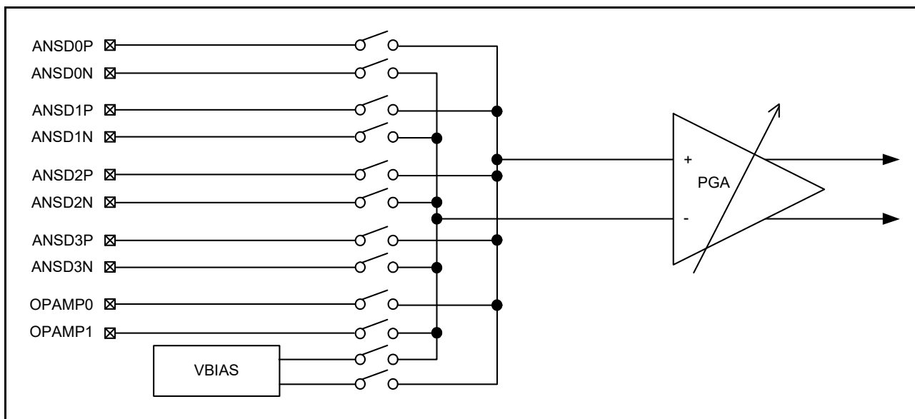
図 33.6 入力マルチプレクサのブロック図
