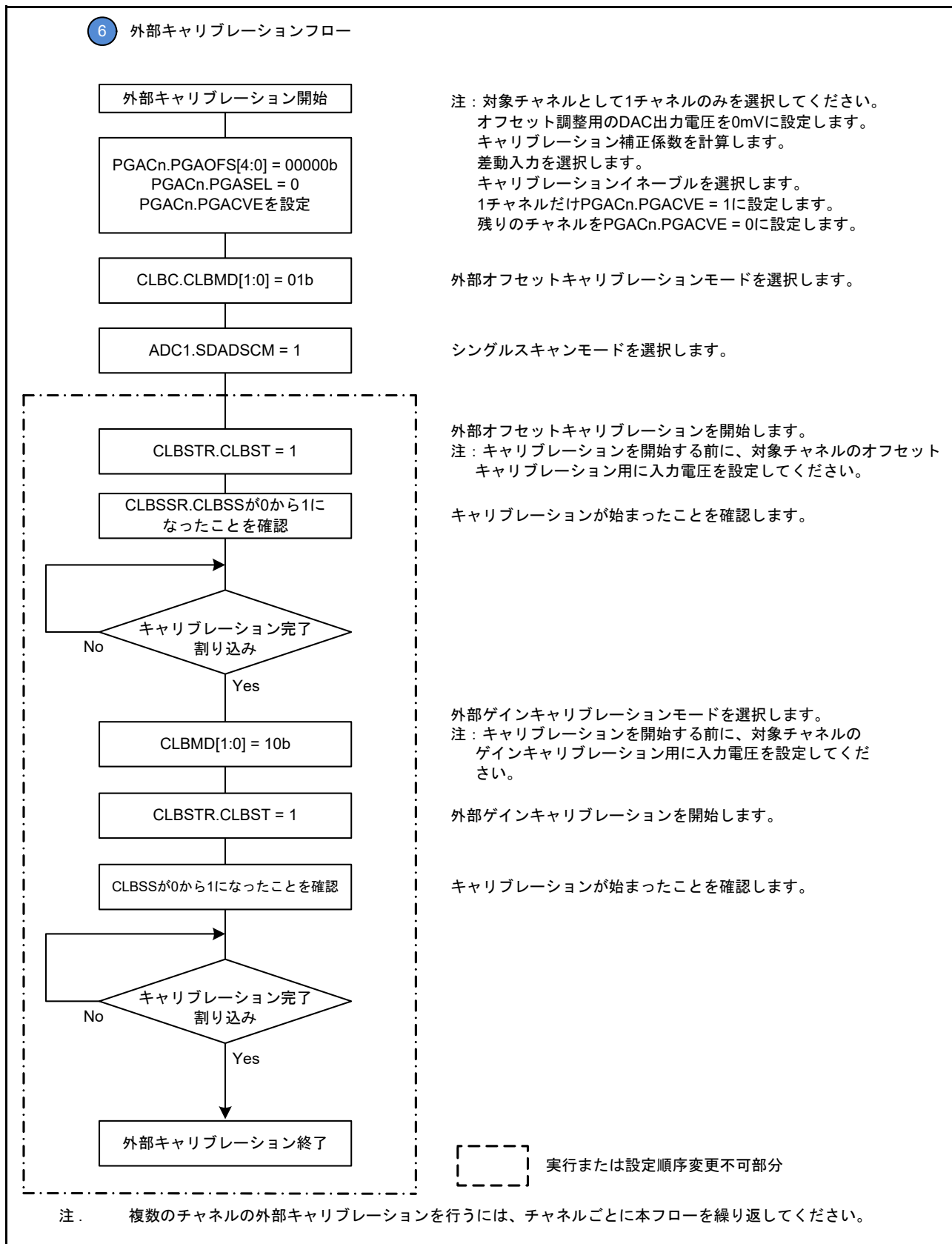
図 33.28 外部キャリブレーションフロー
