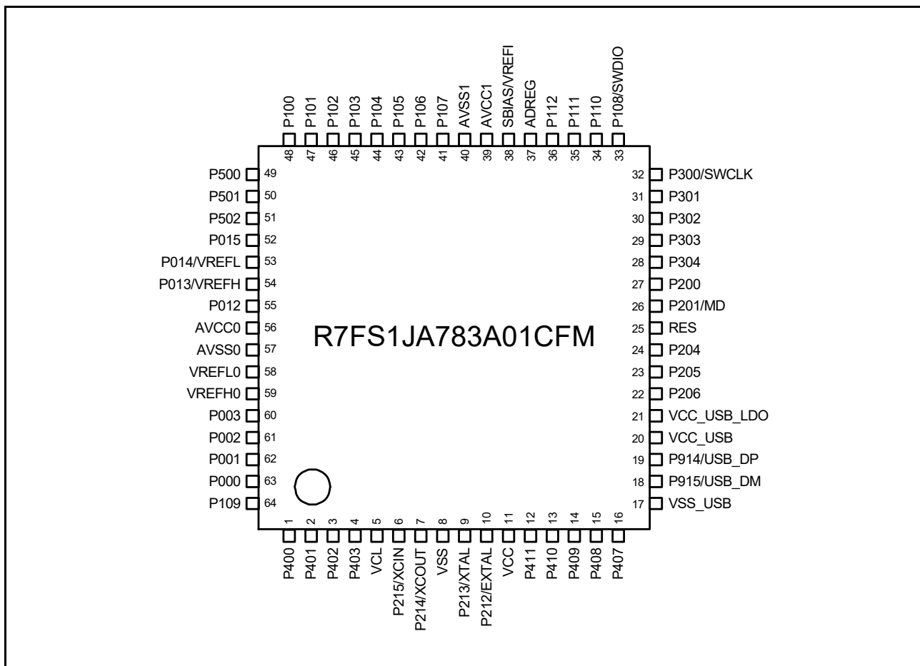
図 1.3 64-pin LQFP のピン配置
