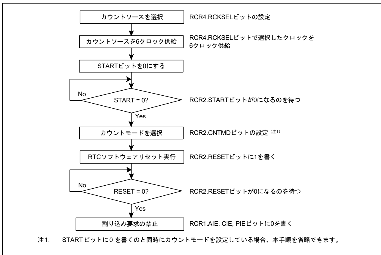
図 23.12 初期化手順
