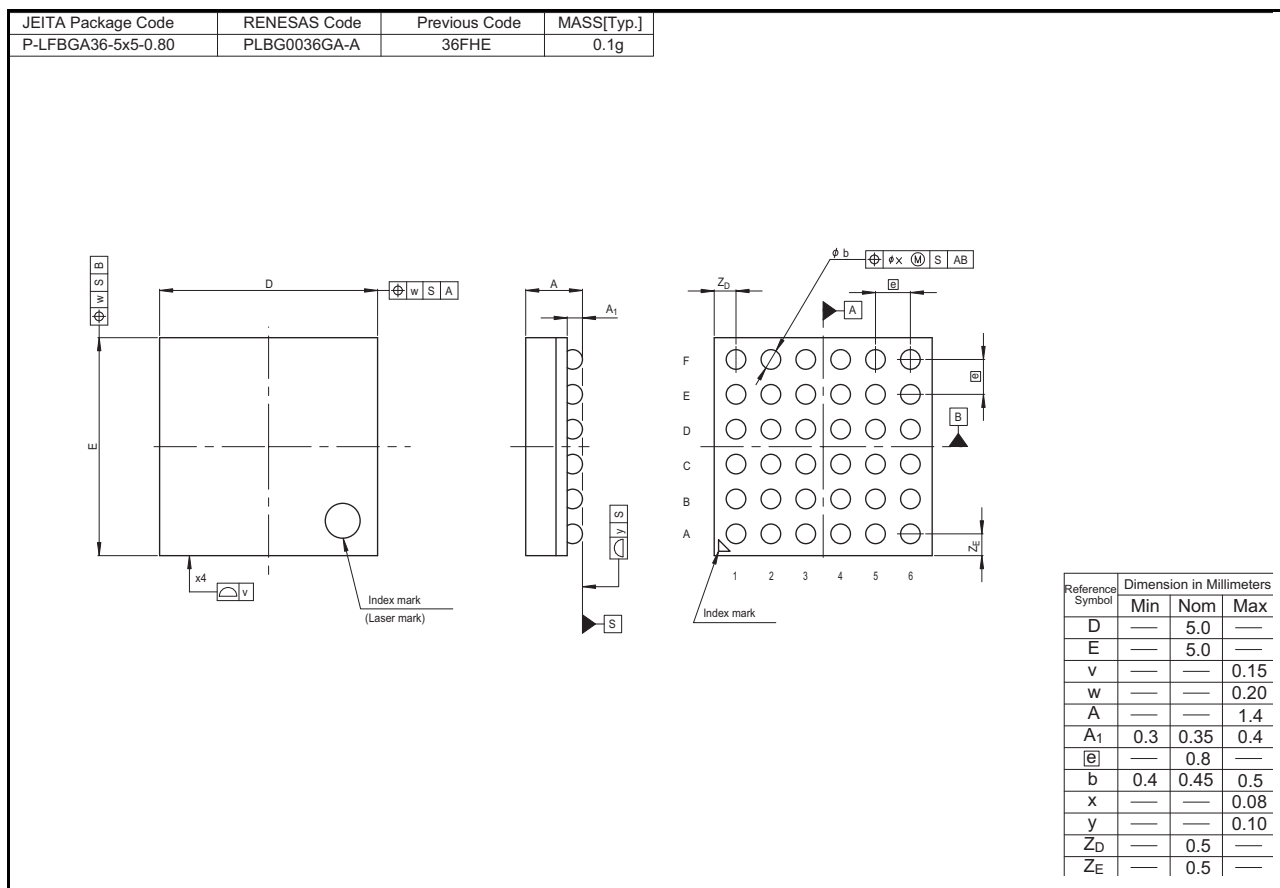
図 2.3 BGA 36 ピン
