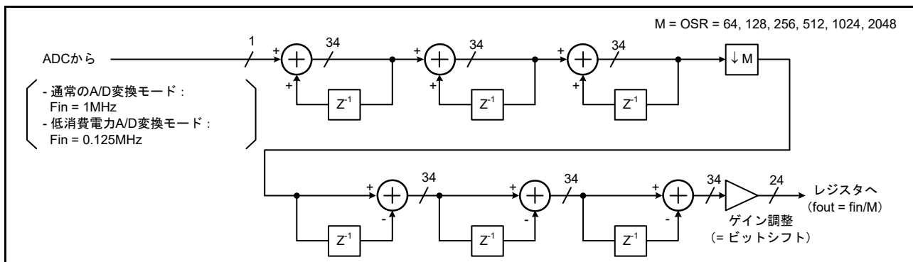
図 33.17 デジタルフィルタのブロック図
