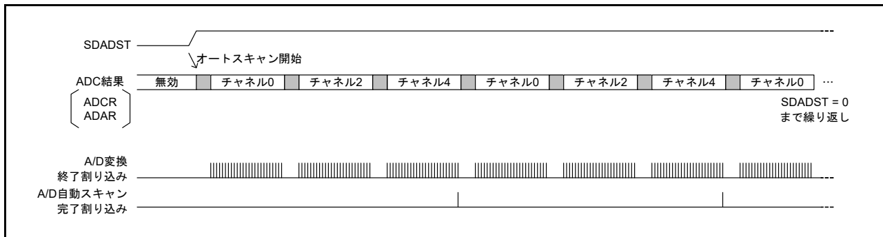
図 33.13 変換チャンネルのスキップ例
