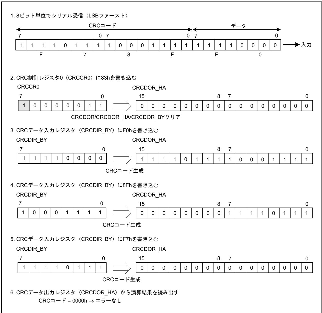
図 31.4 LSB ファーストのデータ受信
