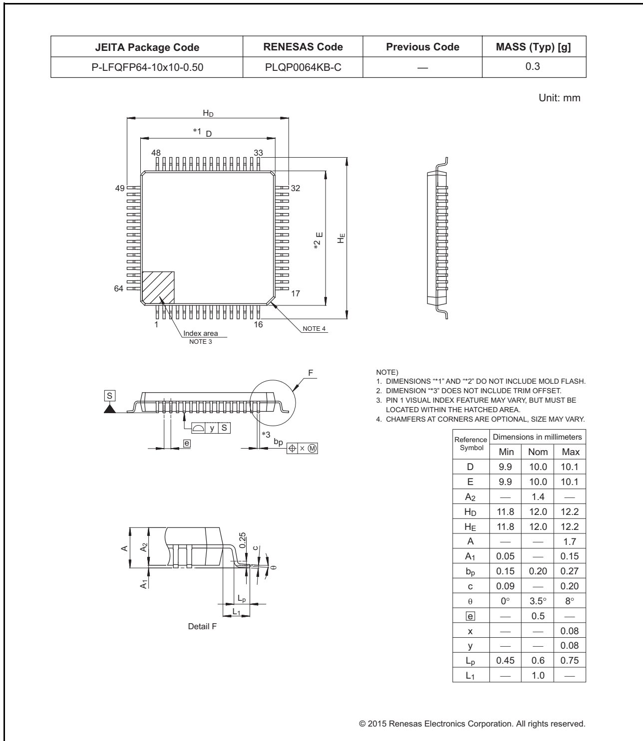
図 2.1 LQFP 64 ピン
