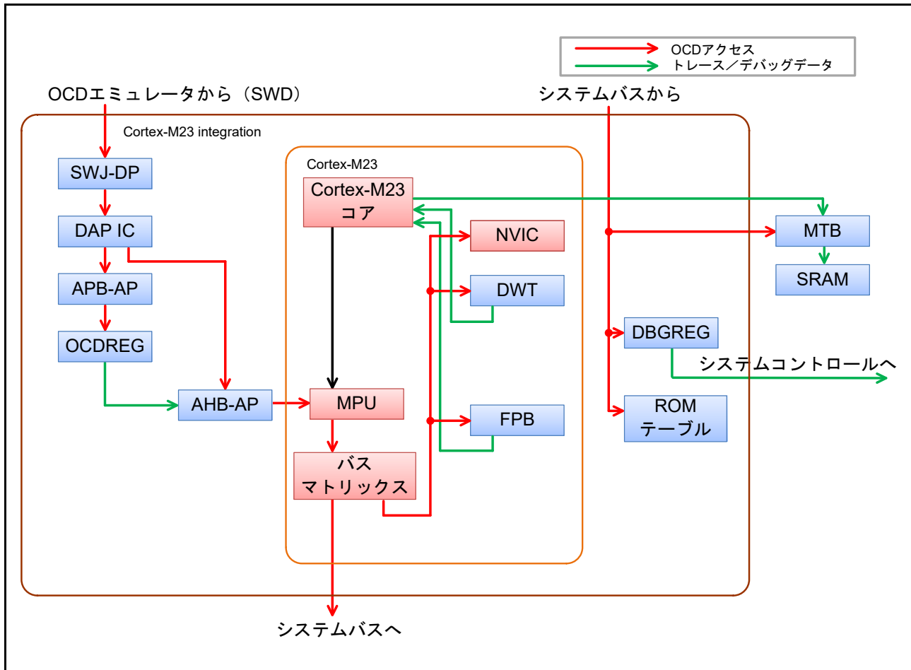
図 2.1 Cortex-M23 CPU ブロック図
