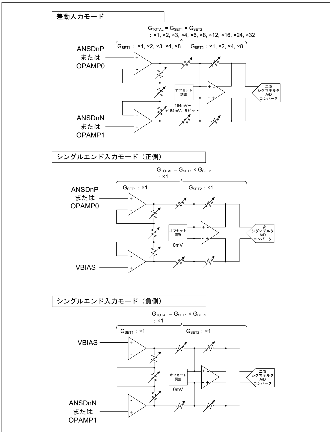
図 33.7 プログラマブルゲイン計装アンプ (PGA)
