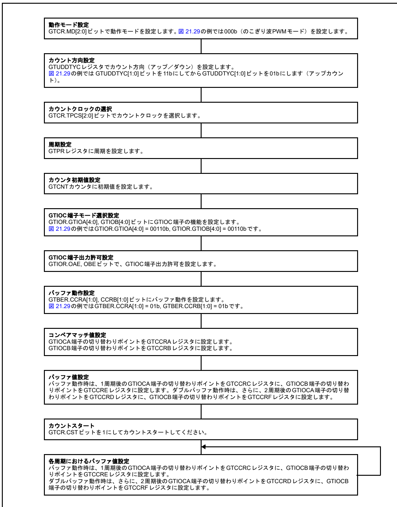
図 21.30 のこぎり波 PWM モード設定例
