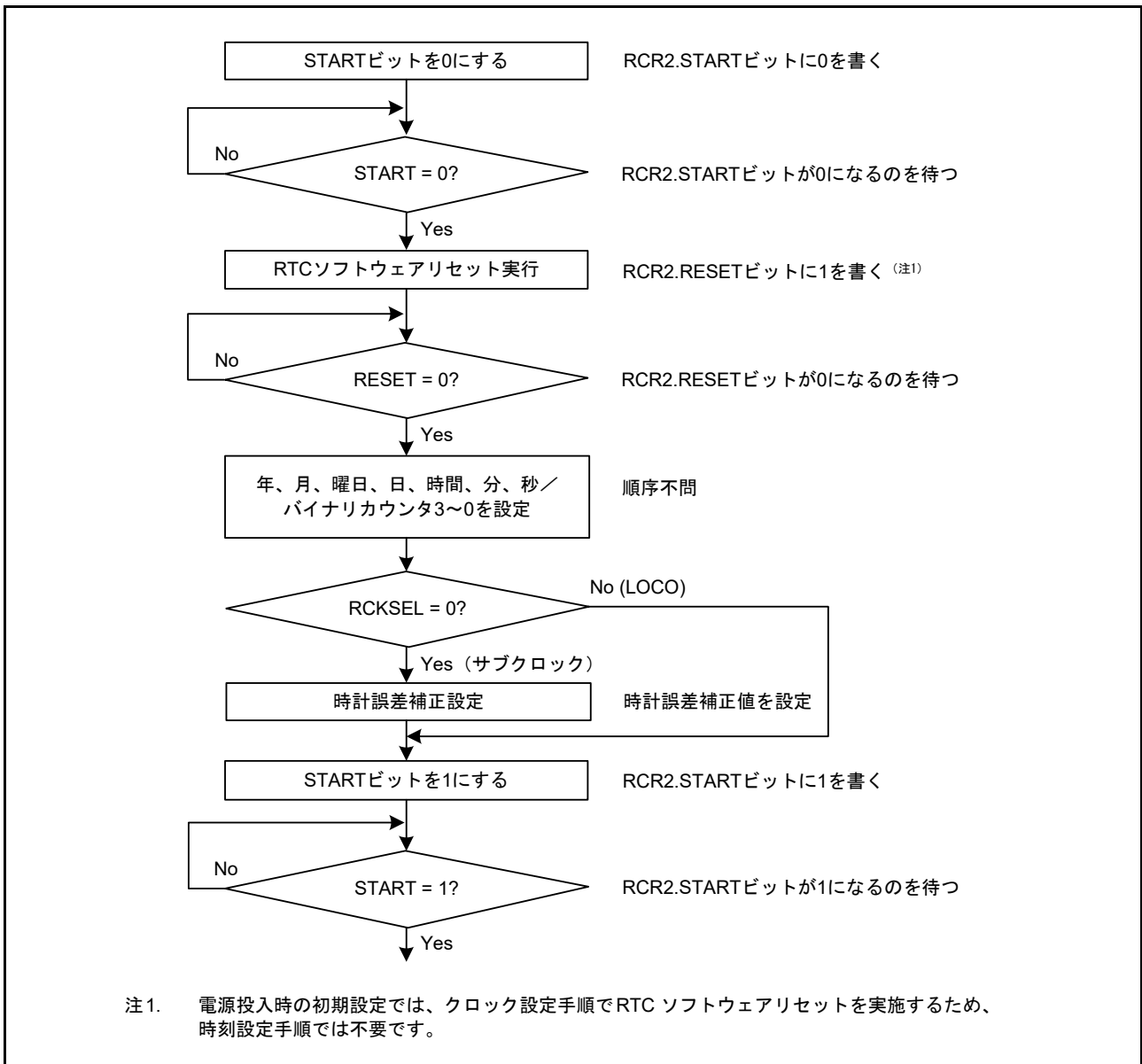
図 23.4 時刻の設定
