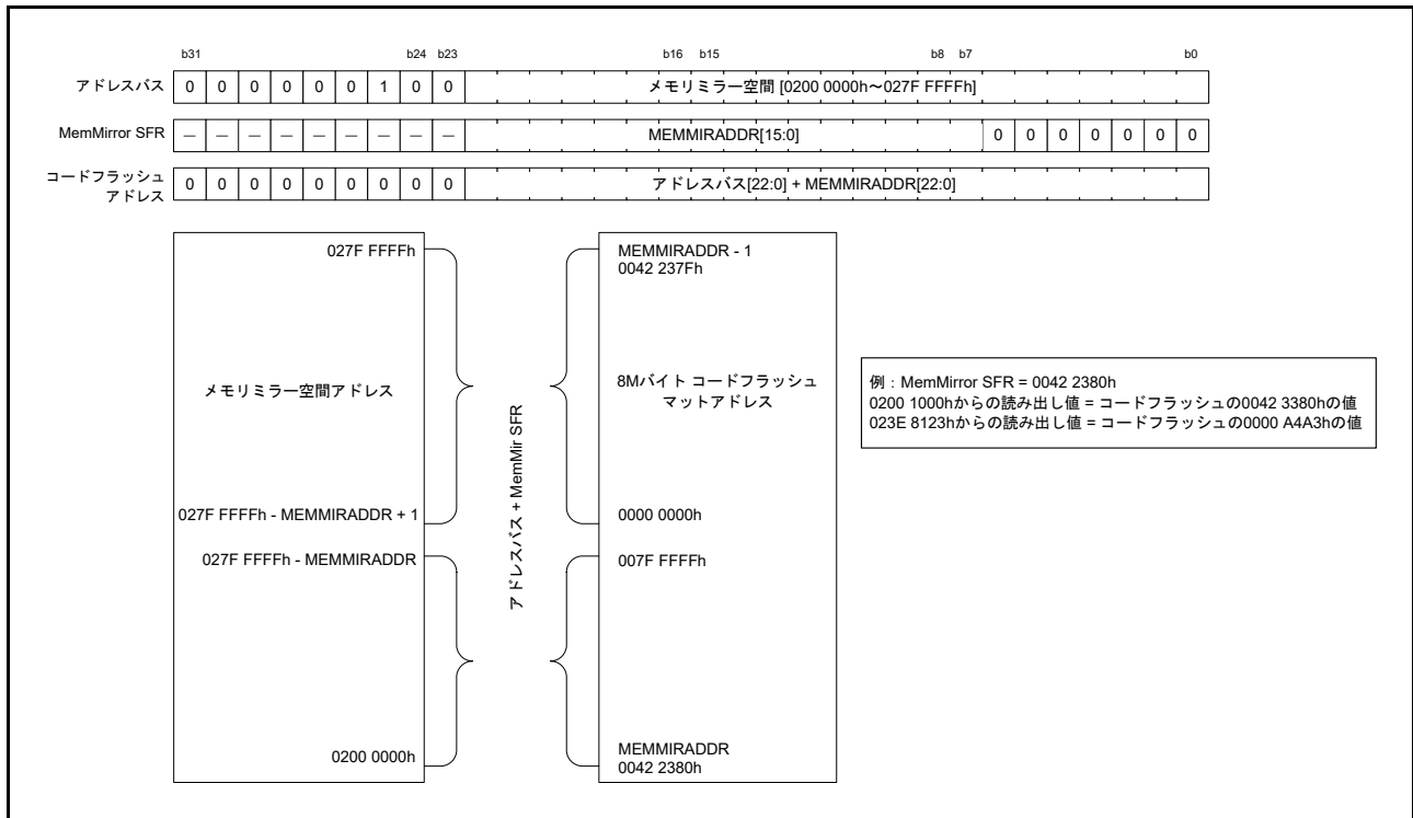
図 5.1 メモリミラー機能動作
