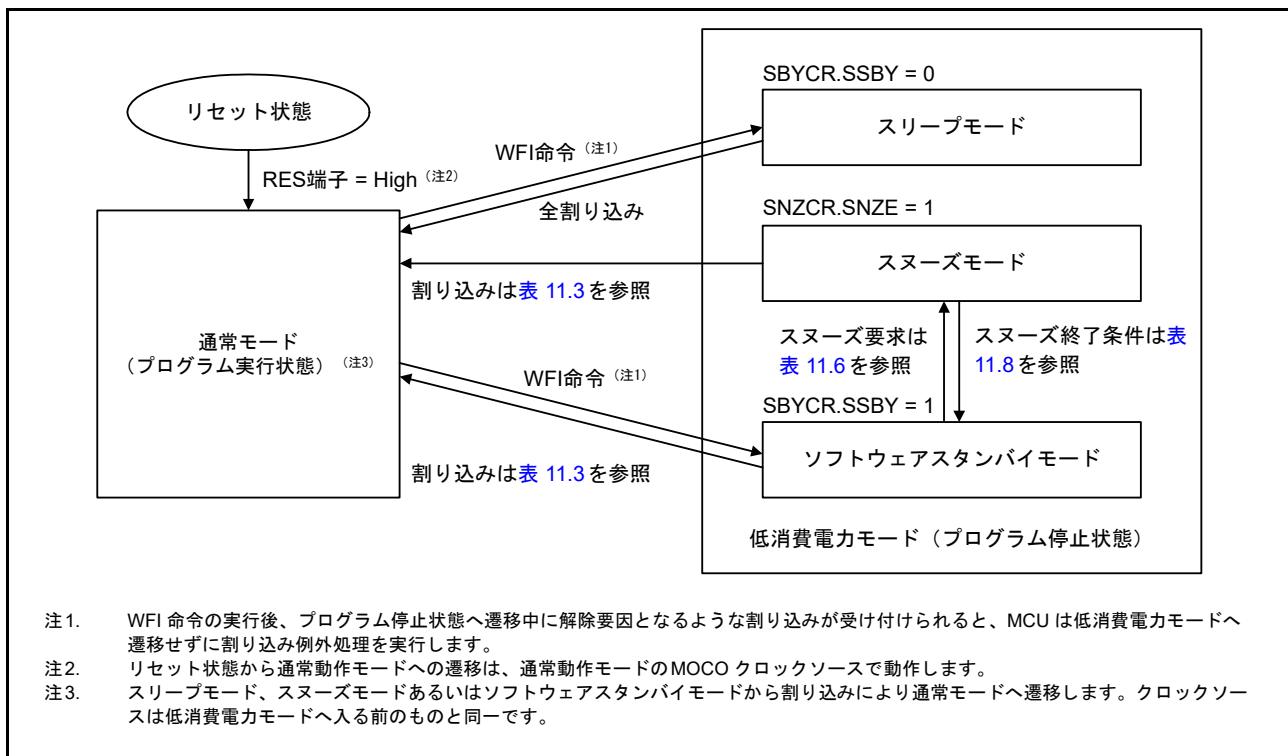
図 11.1 モード遷移
