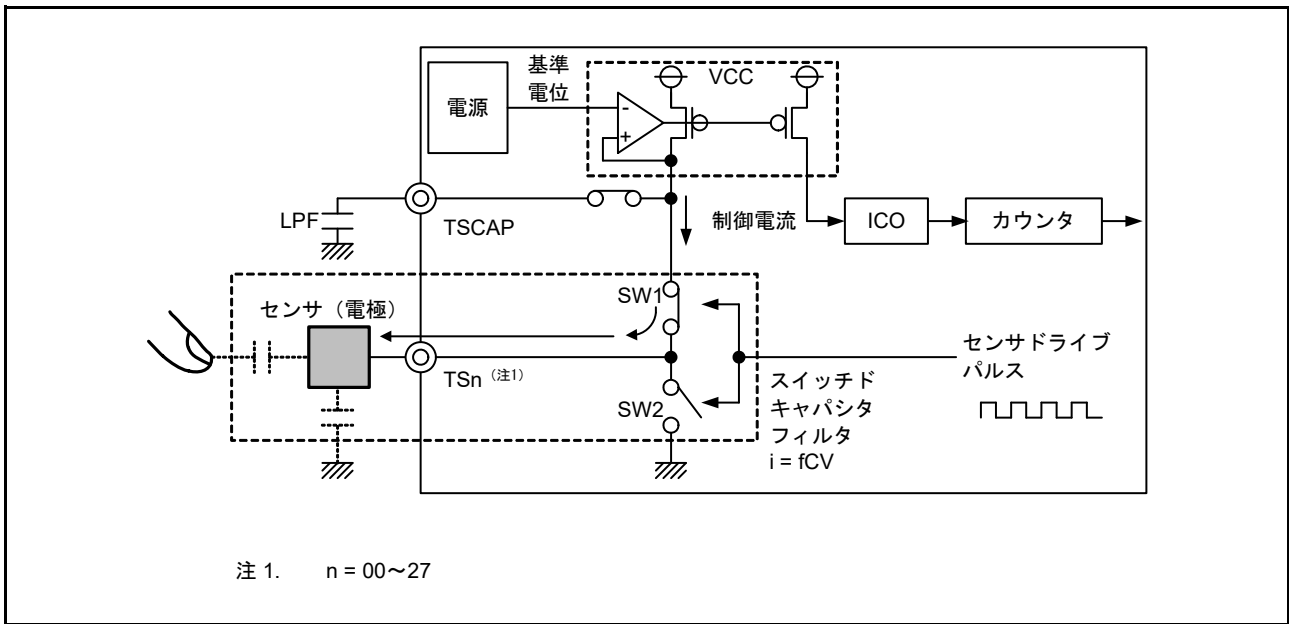
図 40.5 充電動作
