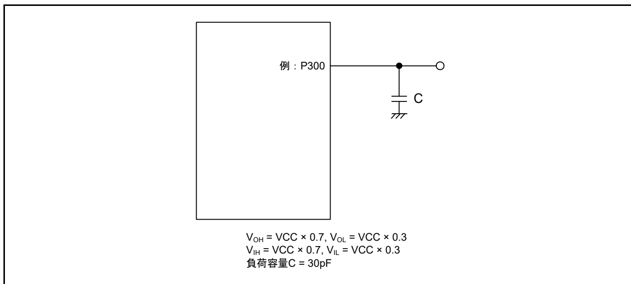
図 47.1 入出力タイミング計測条件
