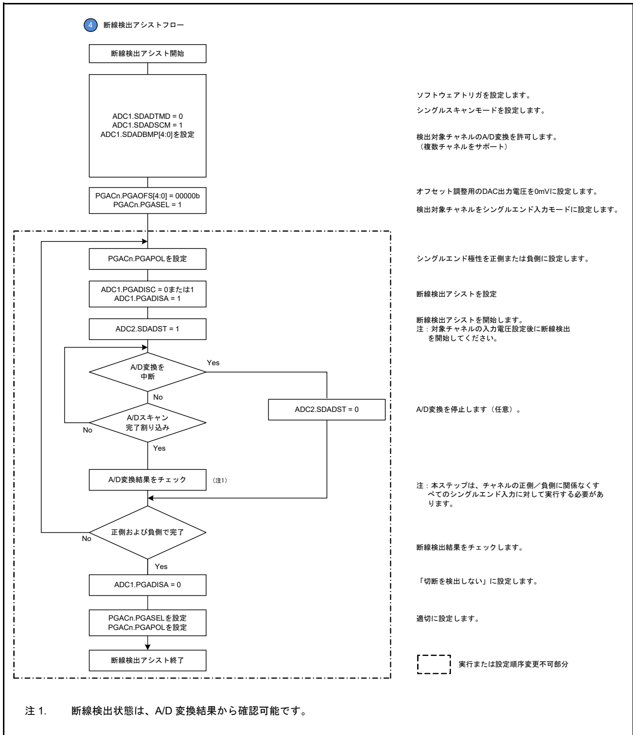
図 33.26 断線検出アシストフロー
