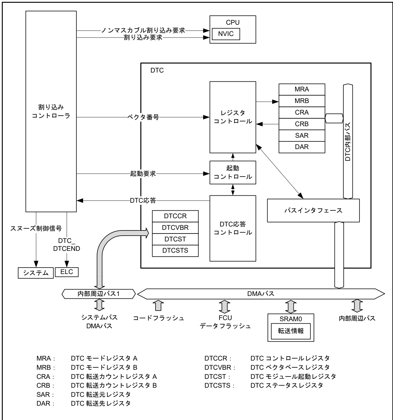
図 16.1 DTC のブロック図
