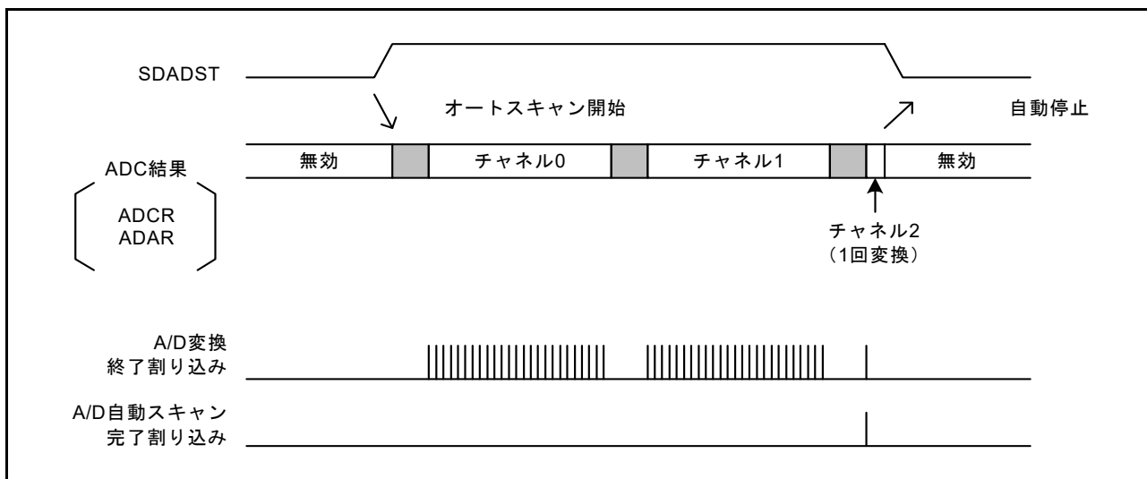
図 33.14 ワンショット動作例
