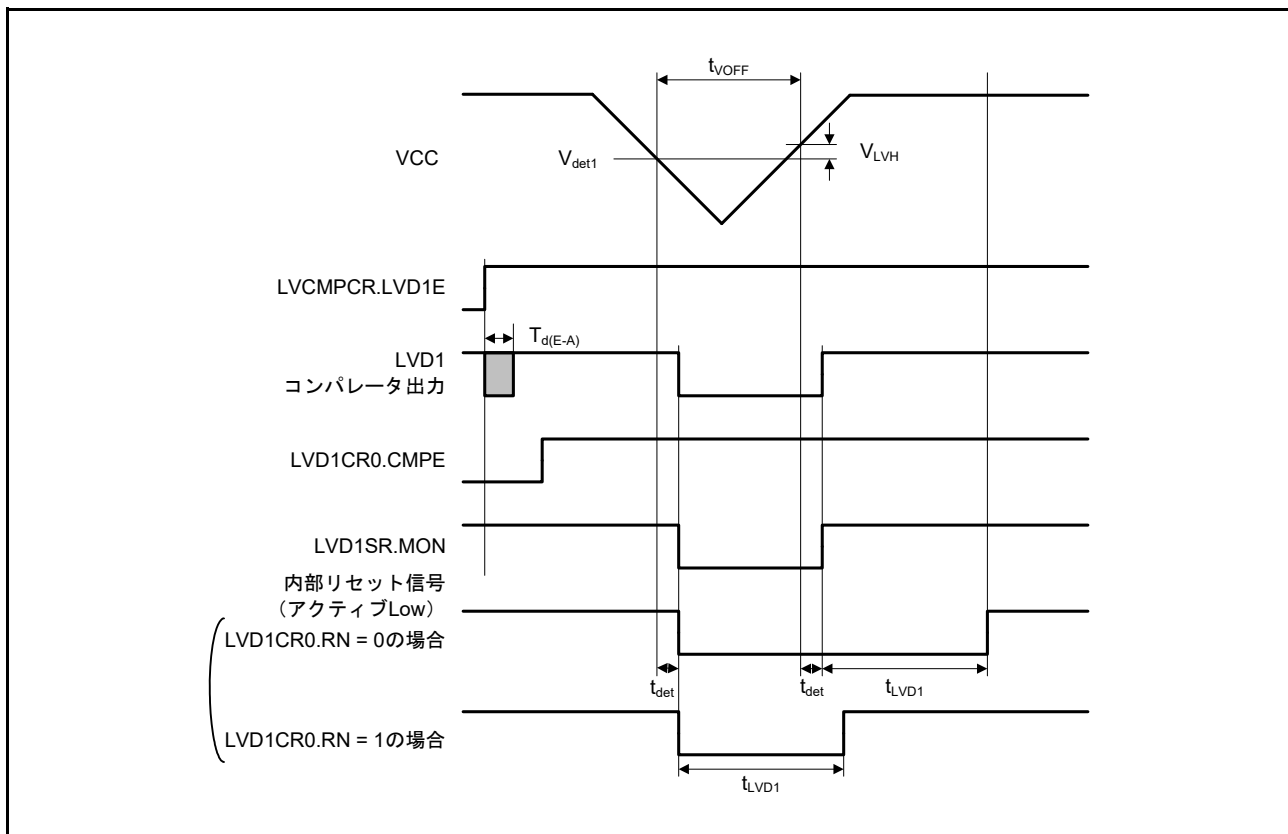
図 47.69 電圧検出回路タイミング ( V_{det1} )
