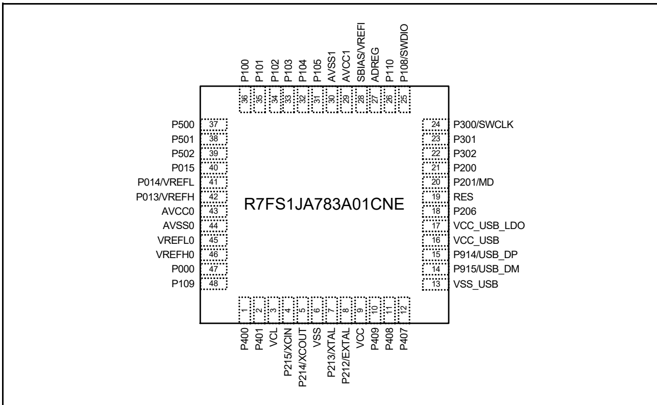
図 1.4 48-pin QFN のピン配置
