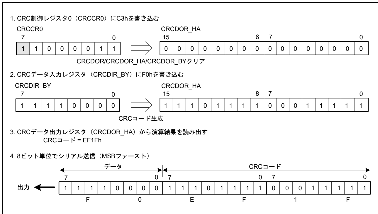
図 31.3 MSB ファーストのデータ送信
