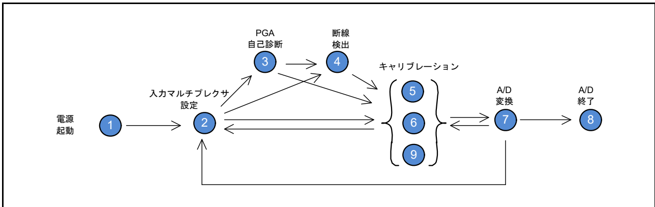
図 33.22 フロー概要
