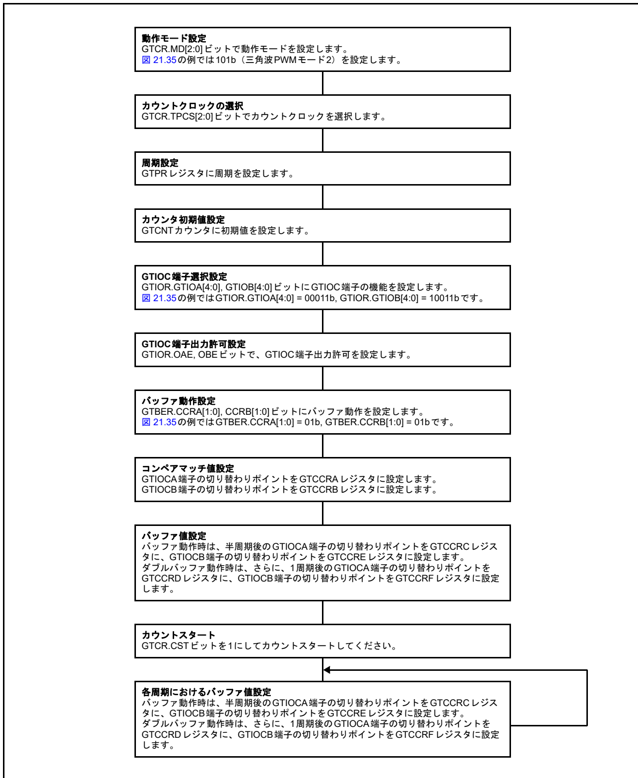
図 21.36 三角波 PWM モード 2 設定例
