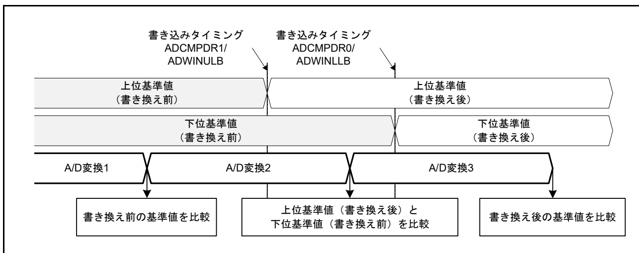
図 32.4 書き換え前後の上側基準値と下側基準値の比較
