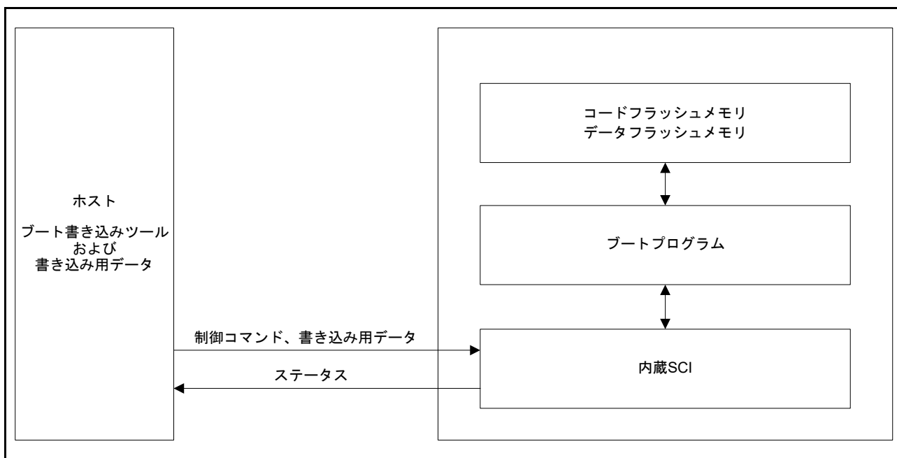
図 43.9 SCI ブートモード時のシステム構成
