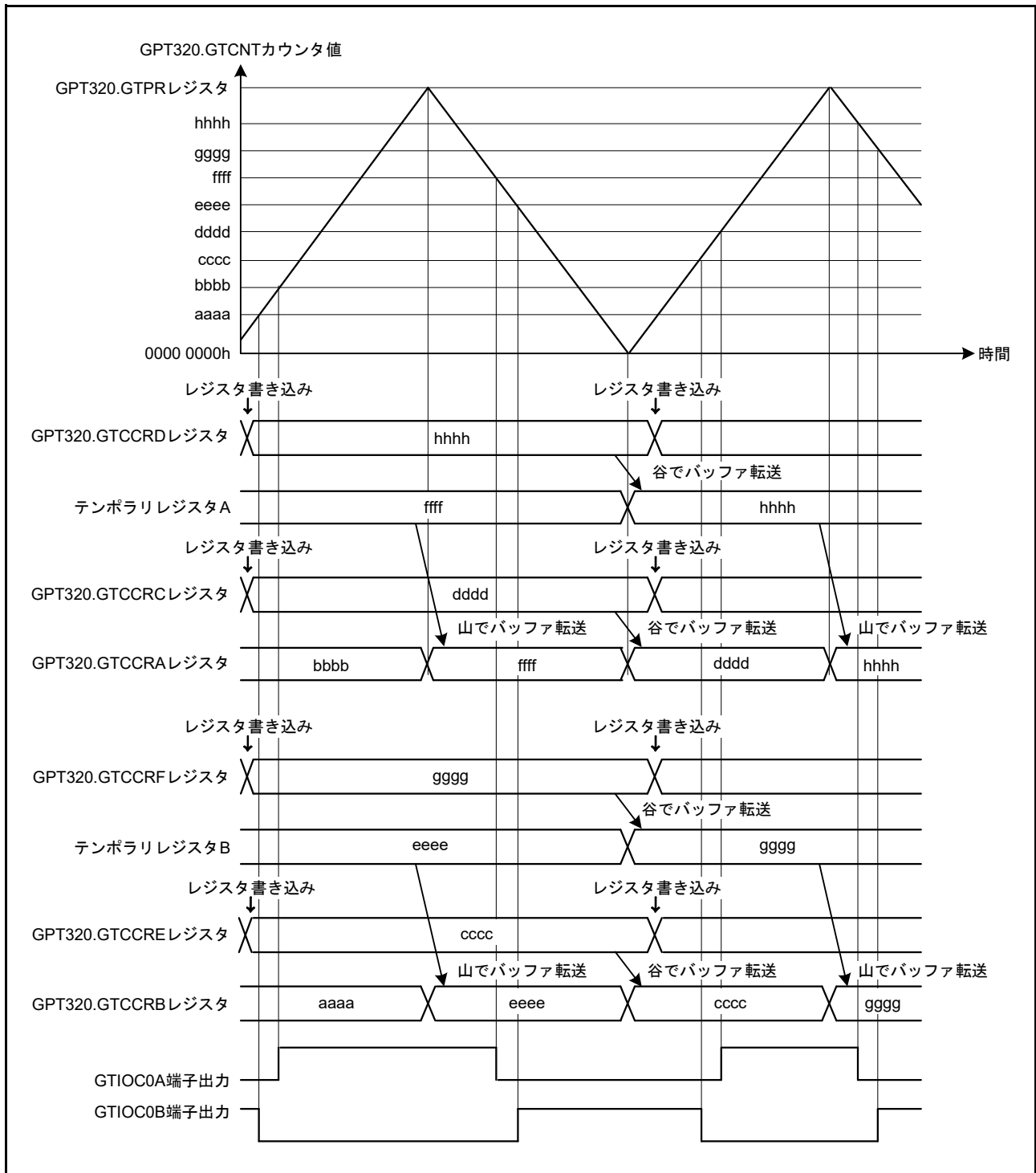
図 21.37 三角波 PWM モード 3 動作例 (カウントスタート時に GTIOC0A 端子 = Low 出力 / GTIOC0B 端子 = High 出力、GTCCRA/GTCCRB レジスタのコンペアマッチ時にトグル出力、周期の終わりで出力保持の場合)
