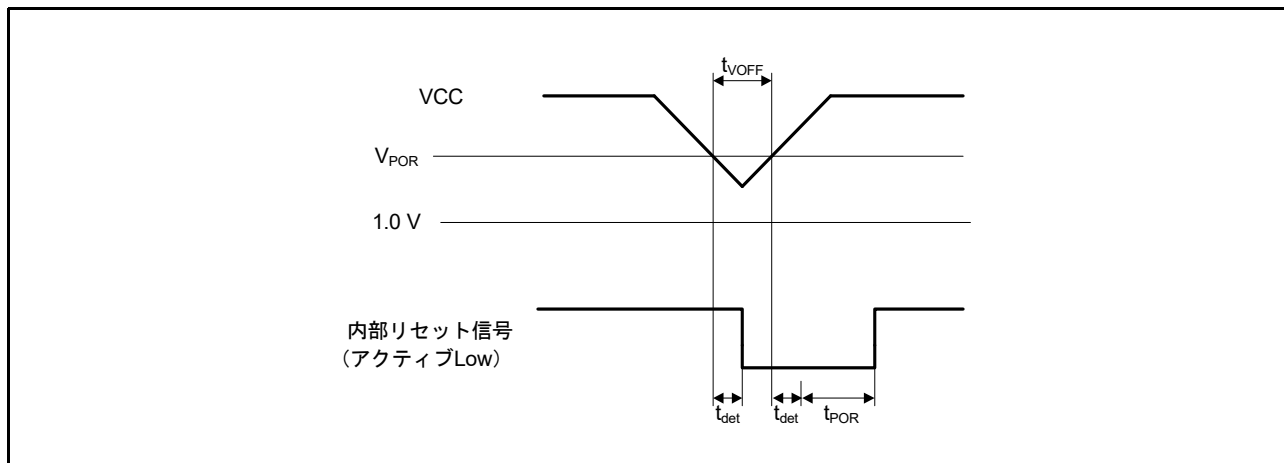
図 47.66 電圧検出リセットタイミング
