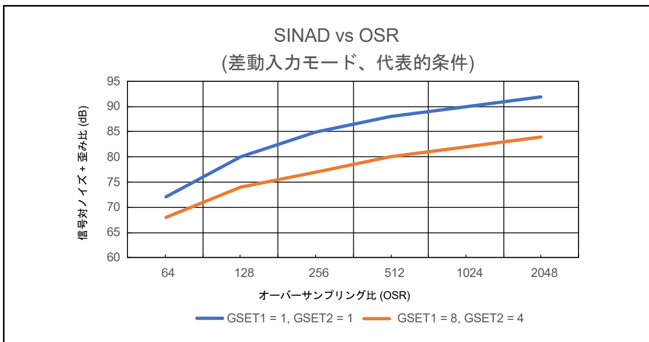
図 47.64 SINAD vs OSR (参考データ)
