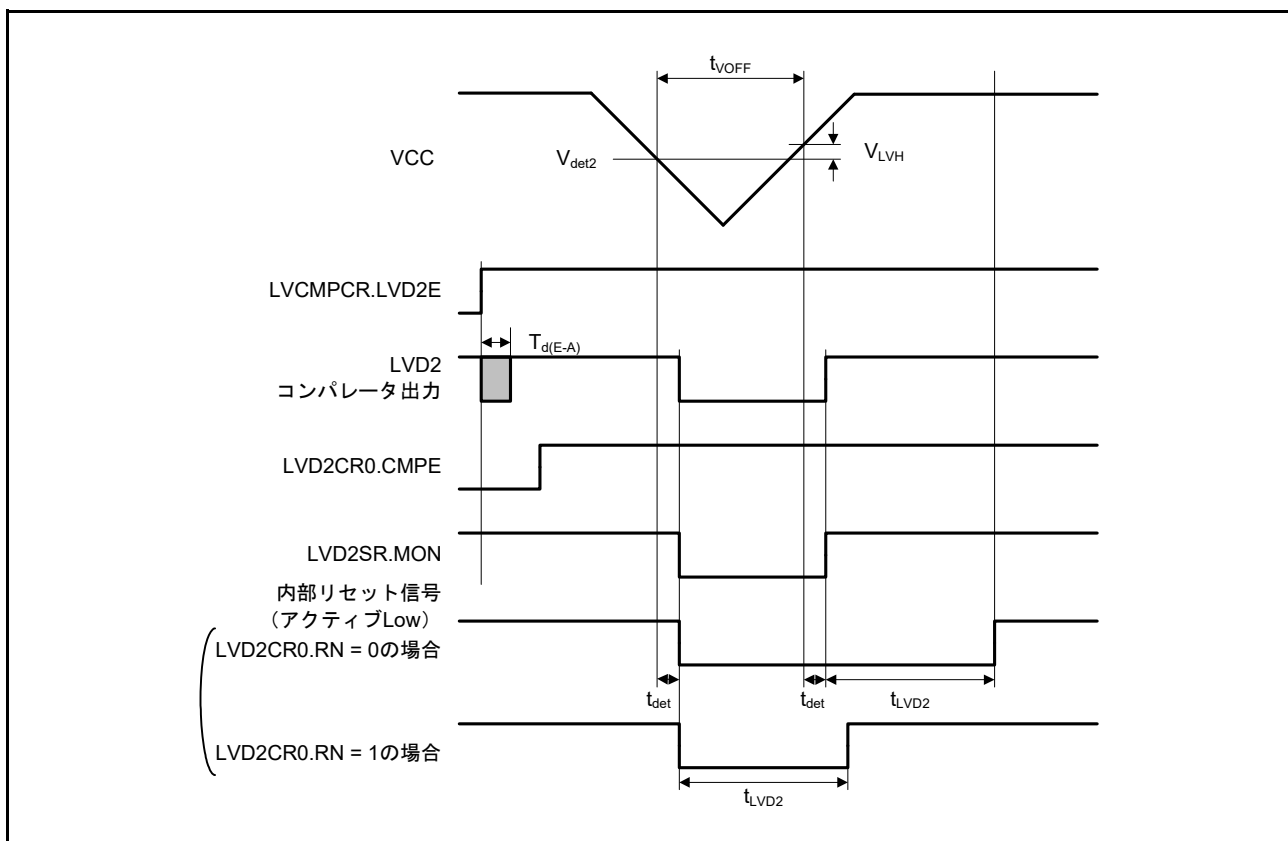
図 47.70 電圧検出回路タイミング ( V_{det2} )
