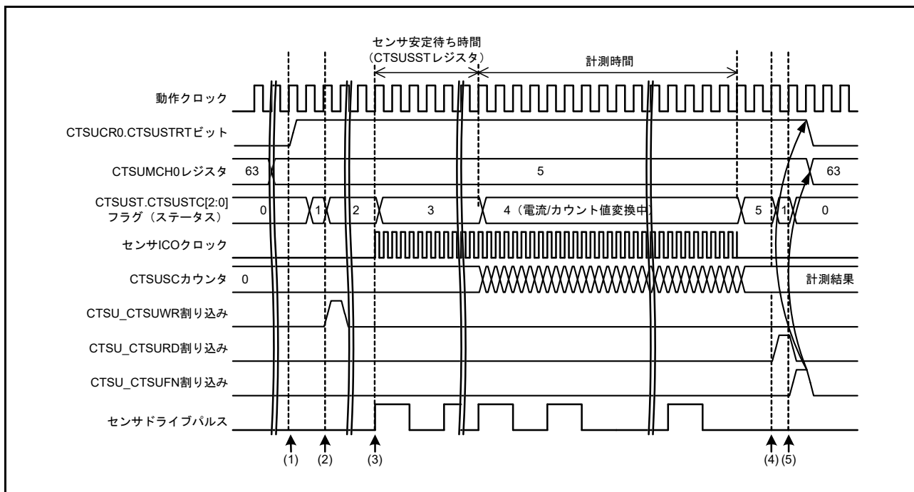
図 40.13 自己容量シングルスキャンモードのタイミング (計測開始条件がソフトウェアトリガの場合)
