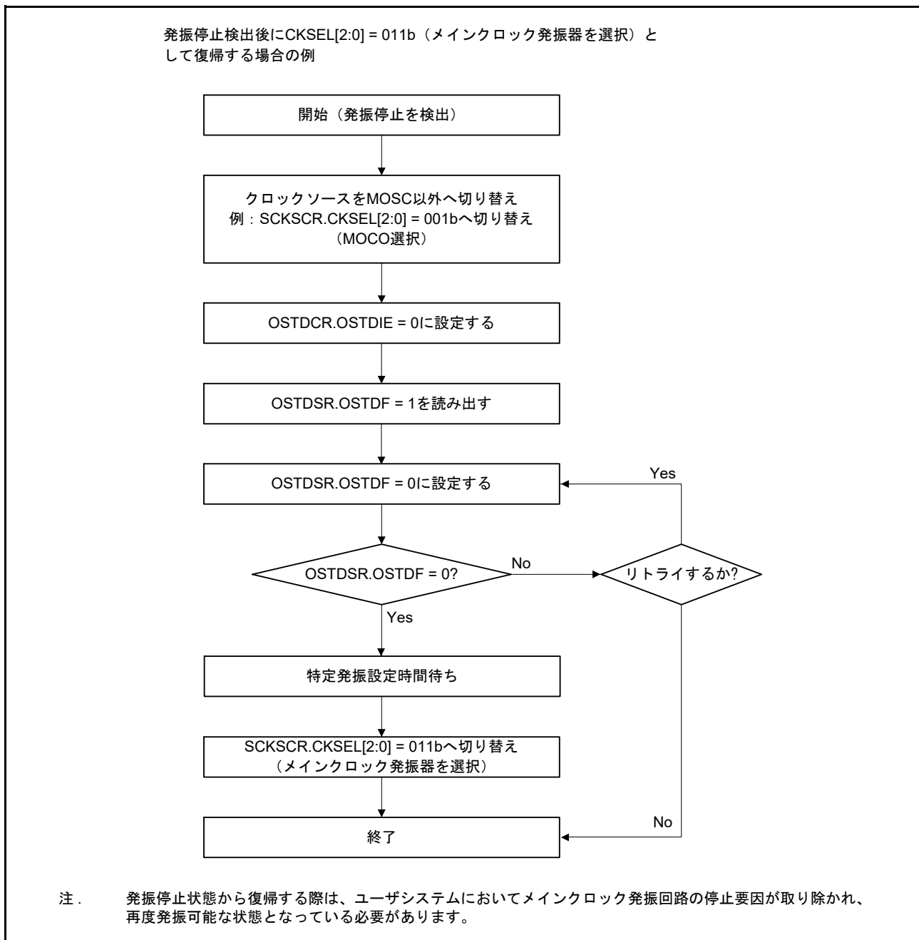
図 9.7 発振停止検出時の復帰フロー
