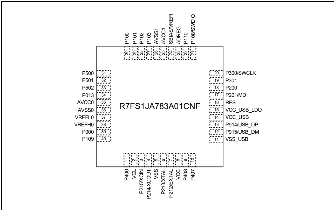
図 1.5 40-pin LQFP のピン配置
