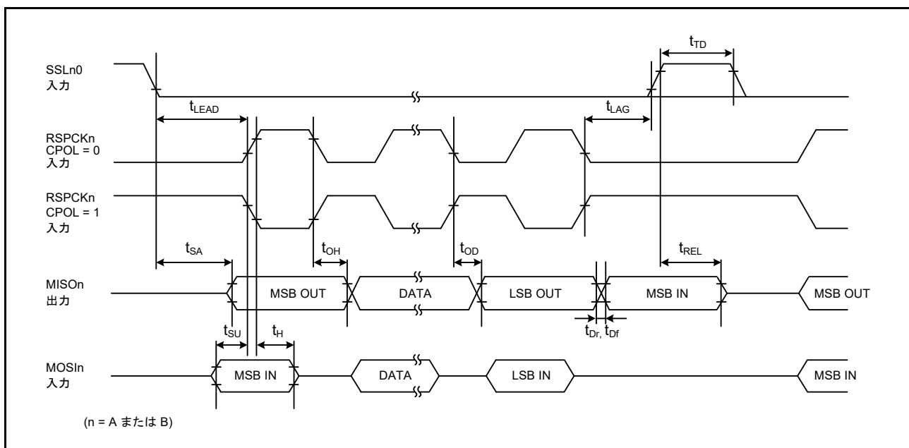
図 47.55 SPI タイミング (スレーブ、CPHA = 0)
