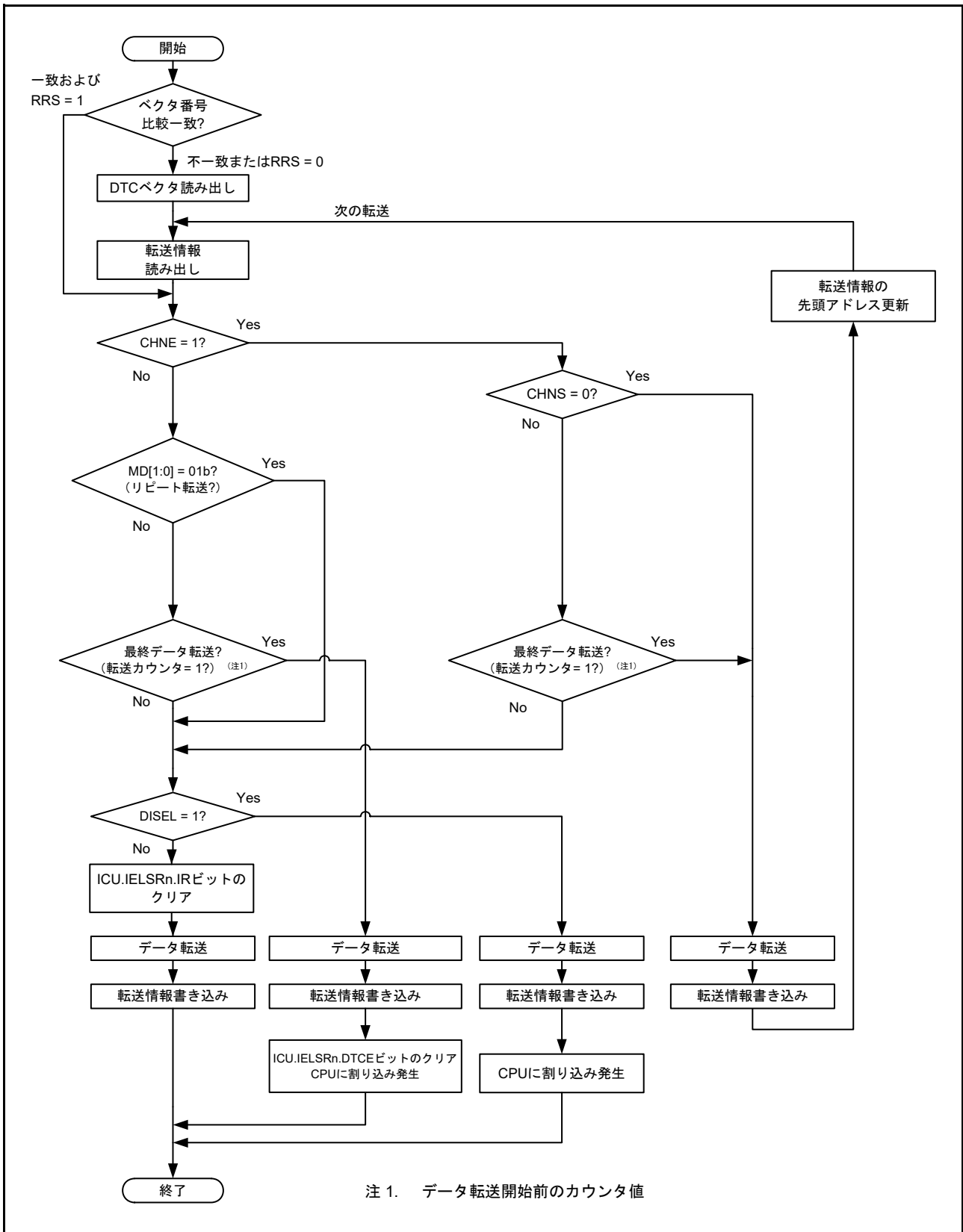
図 16.4 DTC 動作フローチャート
