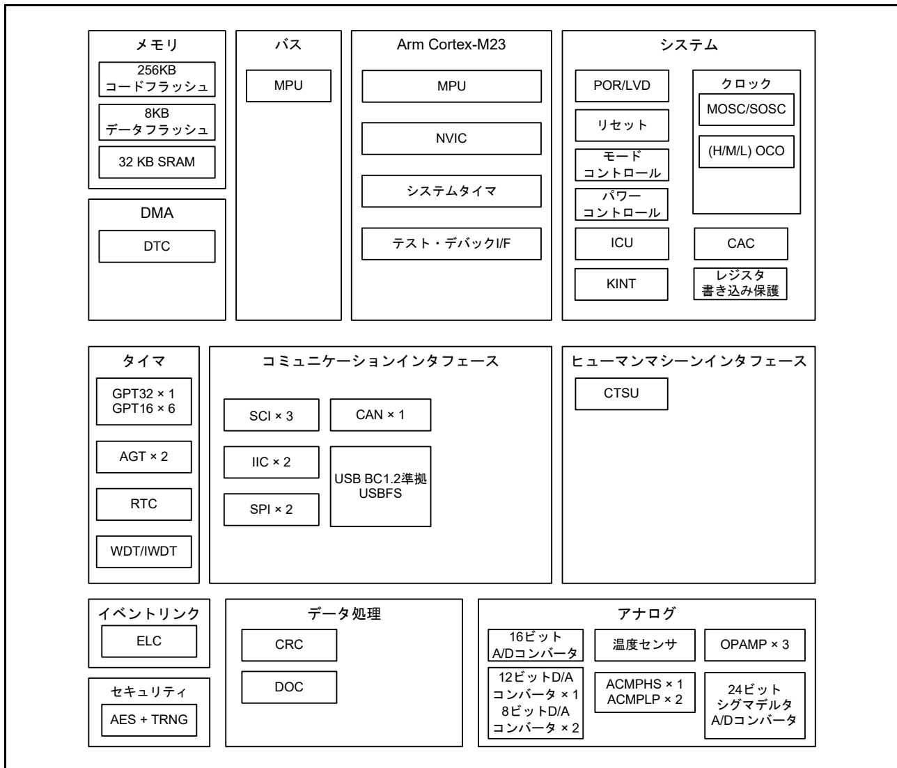
図 1.1 ブロック図
