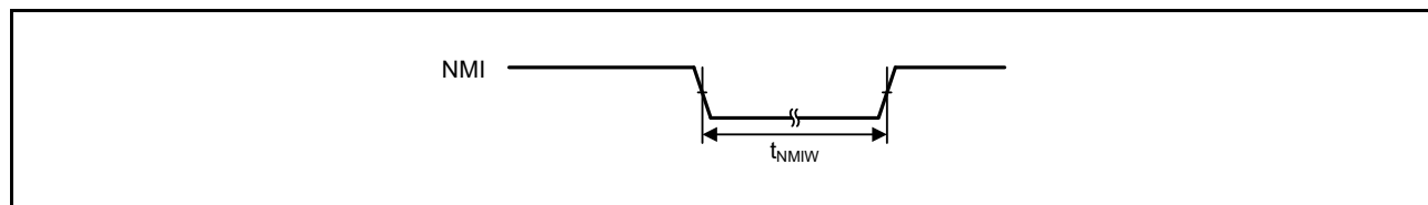
図 47.34 NMI 割り込み入力タイミング
