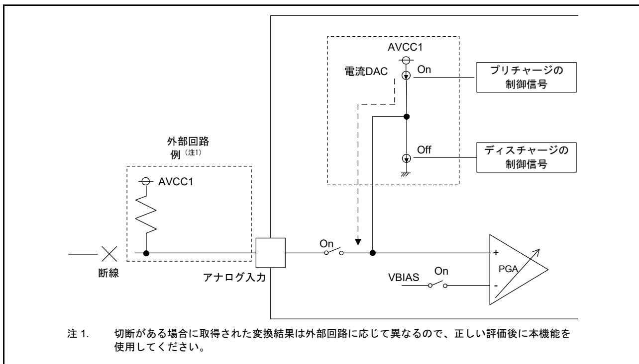
図 33.19 シングルエンド入力モード (正側) でプリチャージ選択時の切断検出例
