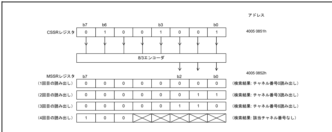
図 29.4 CSSR および MSSR レジスタに対する書き込みと読み出し
