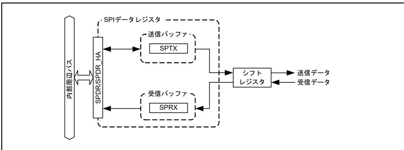
図 30.2 SPDR/SPDR_HA レジスタの構成図
