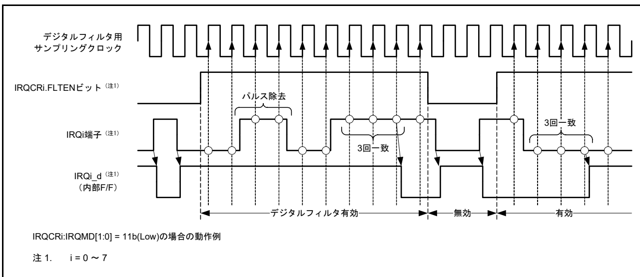
図 13.3 デジタルフィルタの動作例
