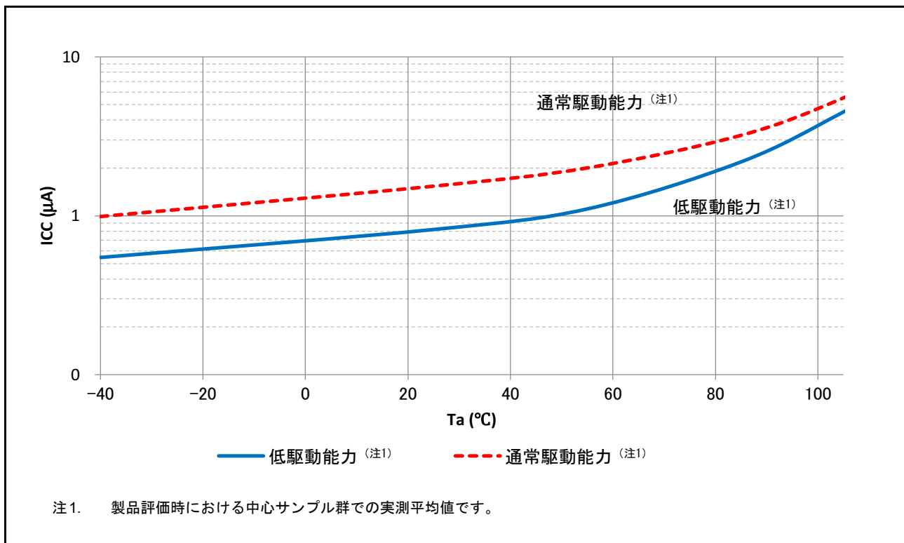
図 47.23 RTC 動作の温度依存性 (参考データ)
