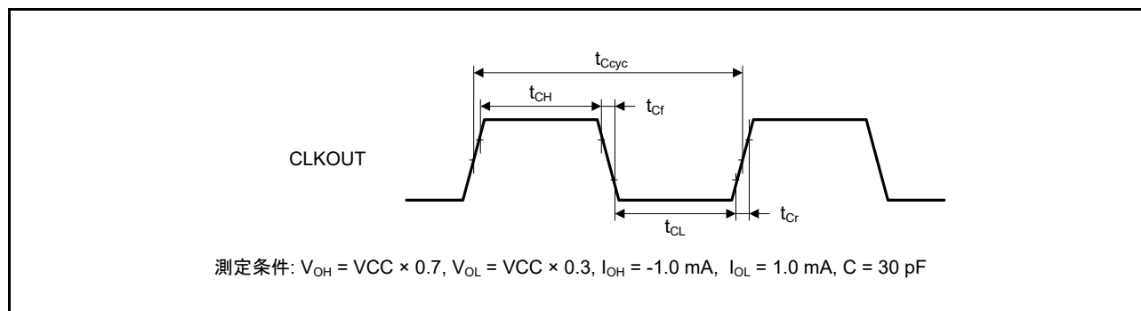
図 47.58 CLKOUT 出力タイミング
