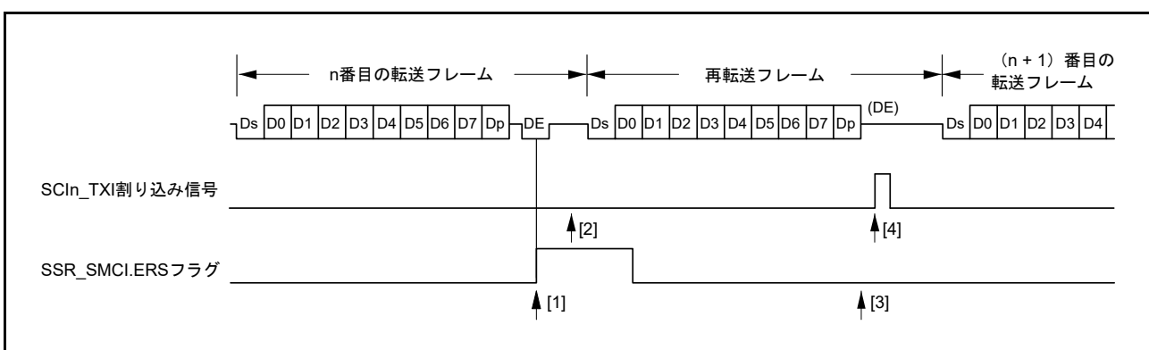
図 27.52 SCI 送信モードでの再転送動作
