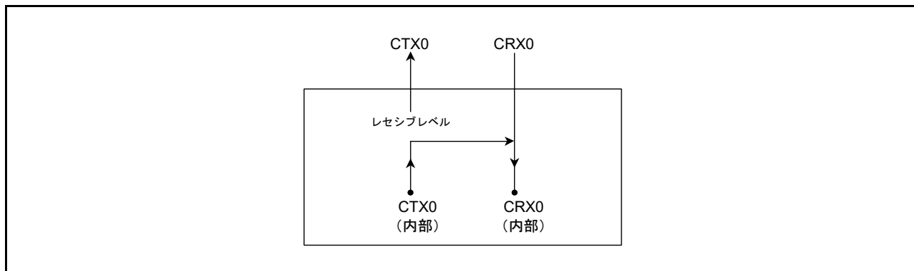
図 29.6 リッスンオンリモード選択時の接続
