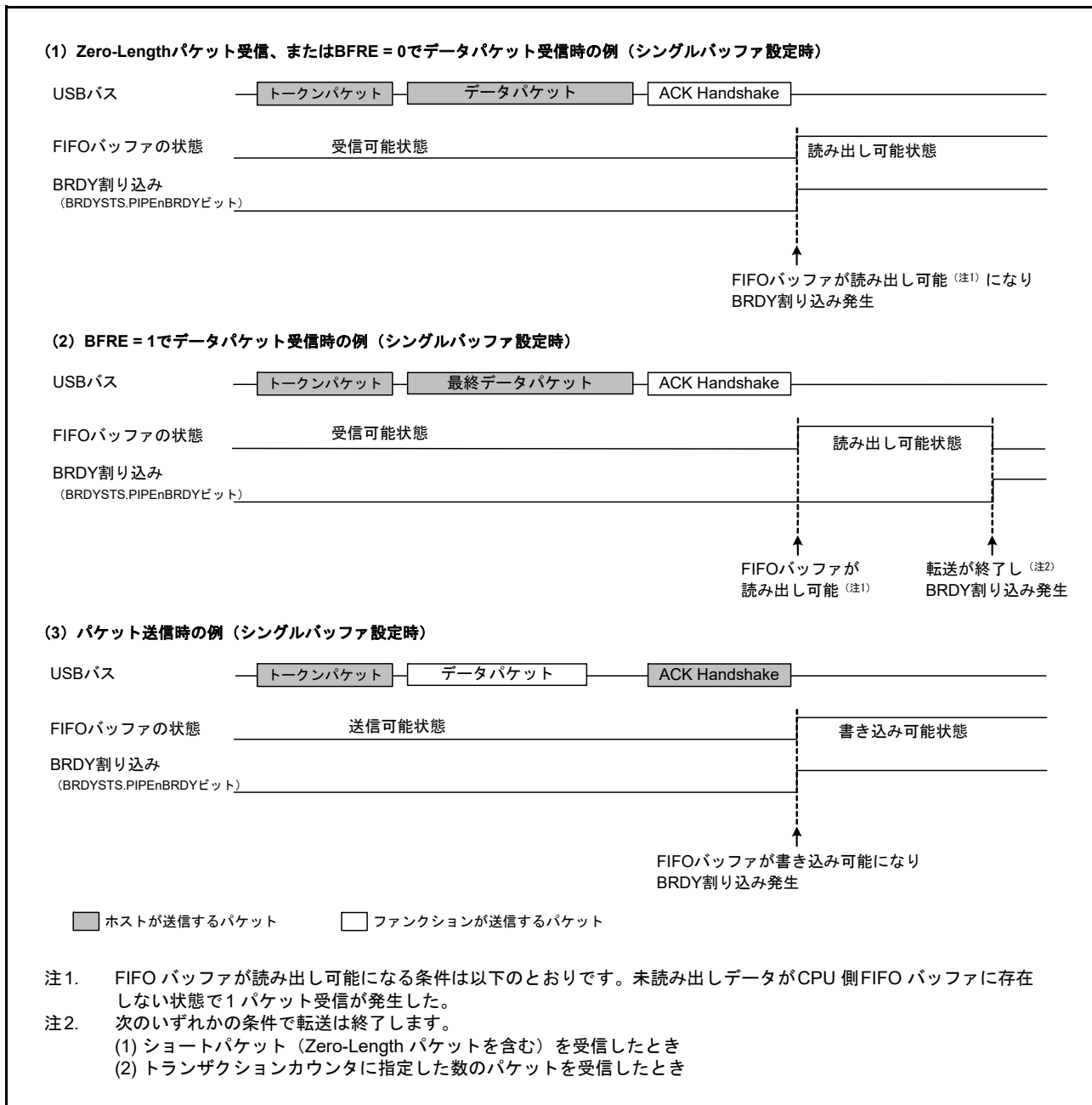
図 26.10 BRDY 割り込み発生タイミング
