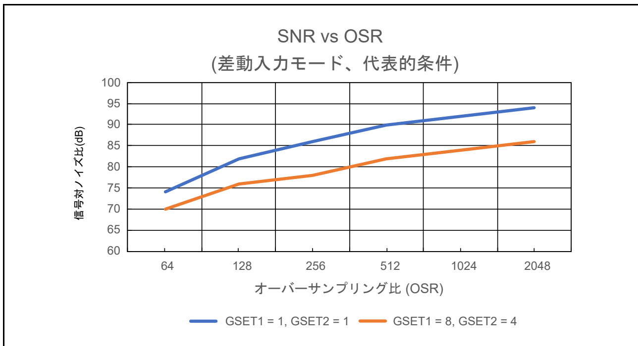
図 47.63 SNR vs OSR (参考データ)
