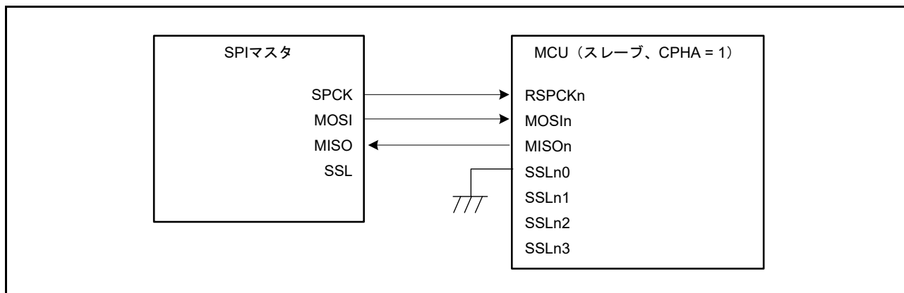
図 30.7 シングルマスタとシングルスレーブの構成例 (MCU はスレーブ、CPHA = 1)
