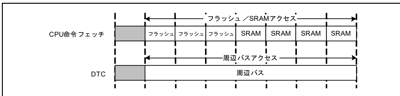
図 14.2 並列動作の例
