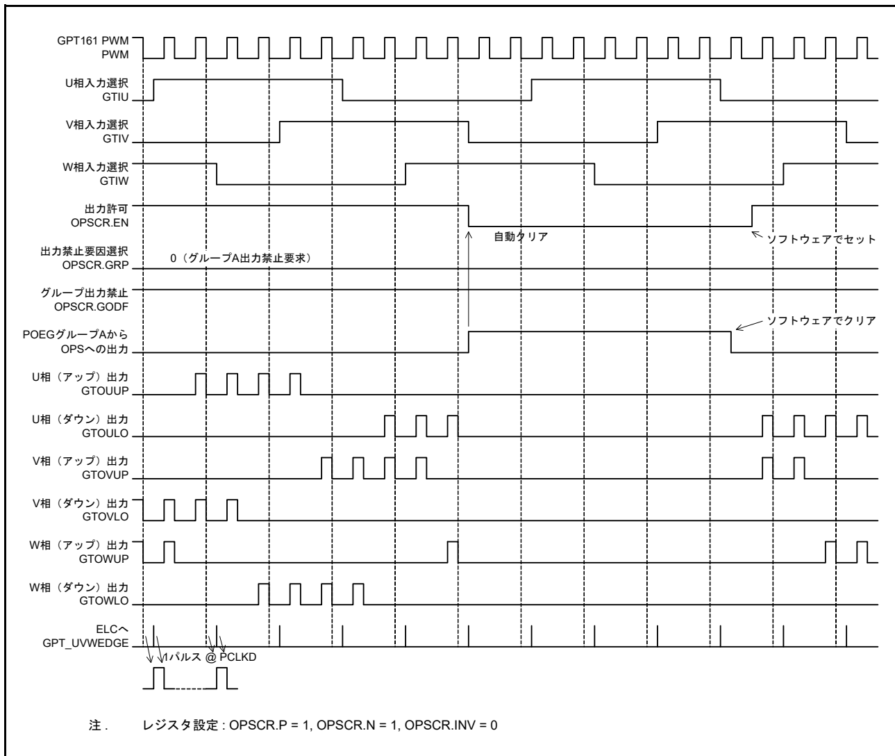
図 21.80 グループ出力禁止制御動作例
