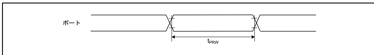
図 47.36 I/Oポート入力タイミング
