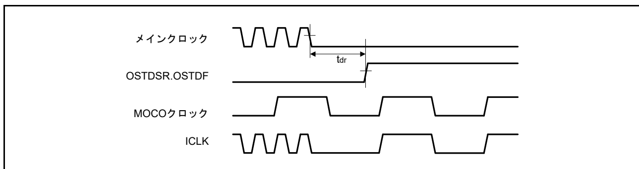
図 47.65 発振停止検出タイミング
