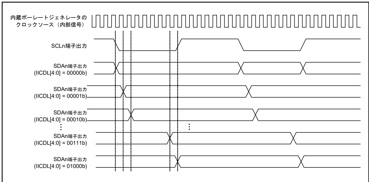
図 27.62 SDA n 出力遅延のタイミング
