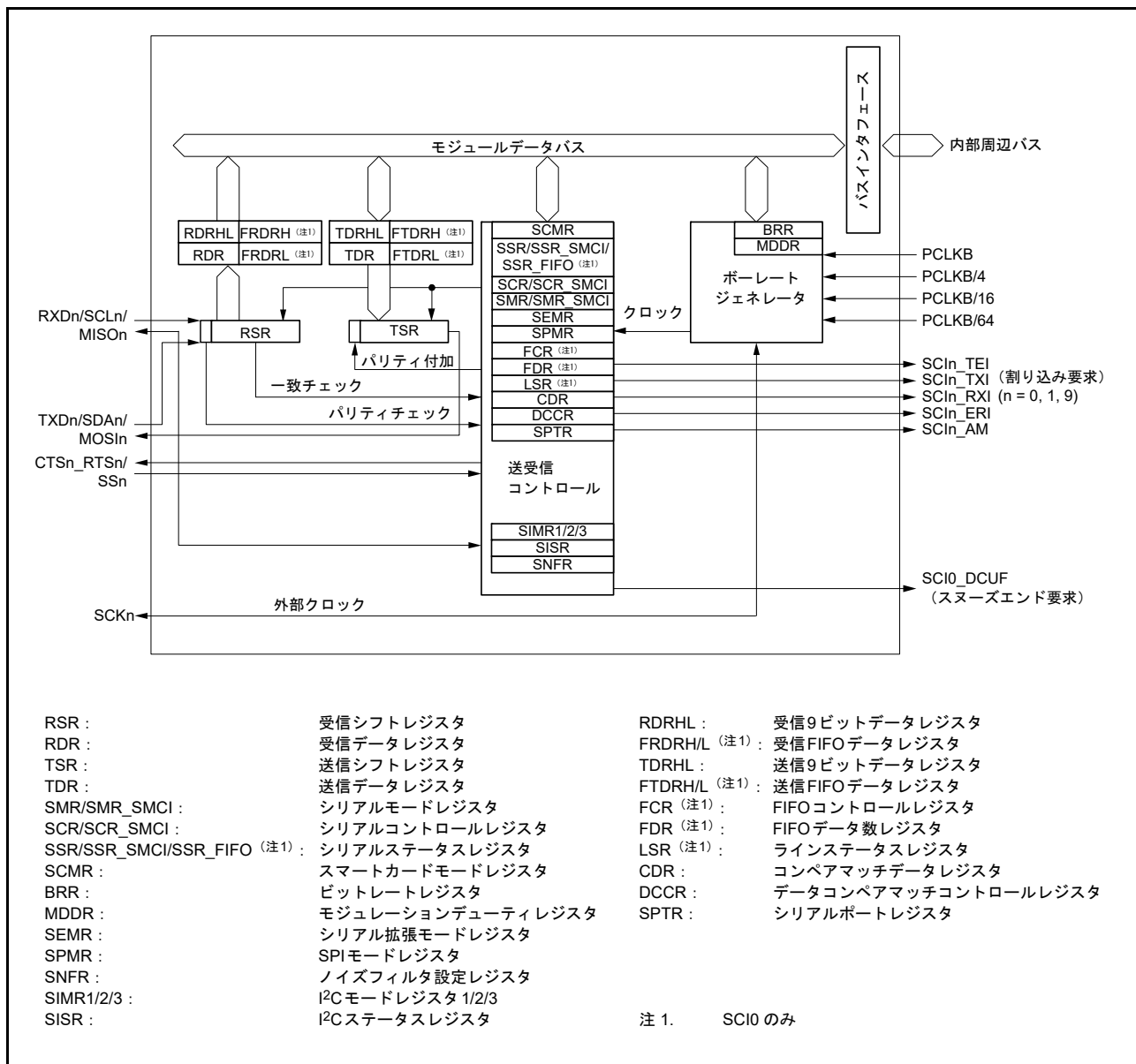
図 27.1 SCIのブロック図
