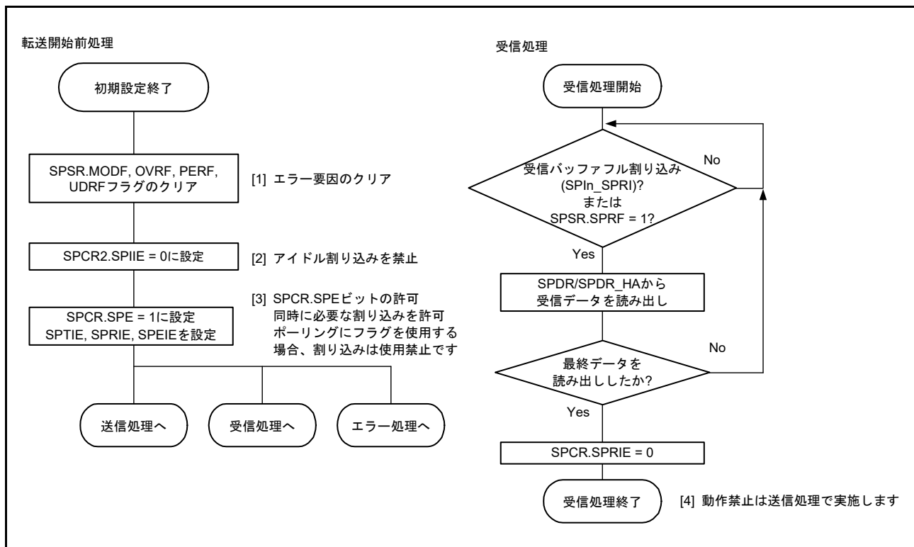
図 30.34 マスタモード時の受信フロー
