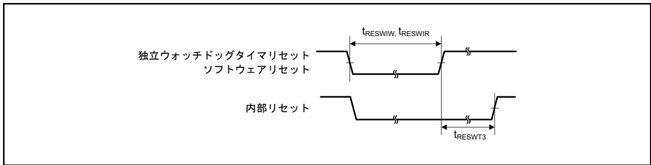
図 47.31 リセット入カタイミング (2)
