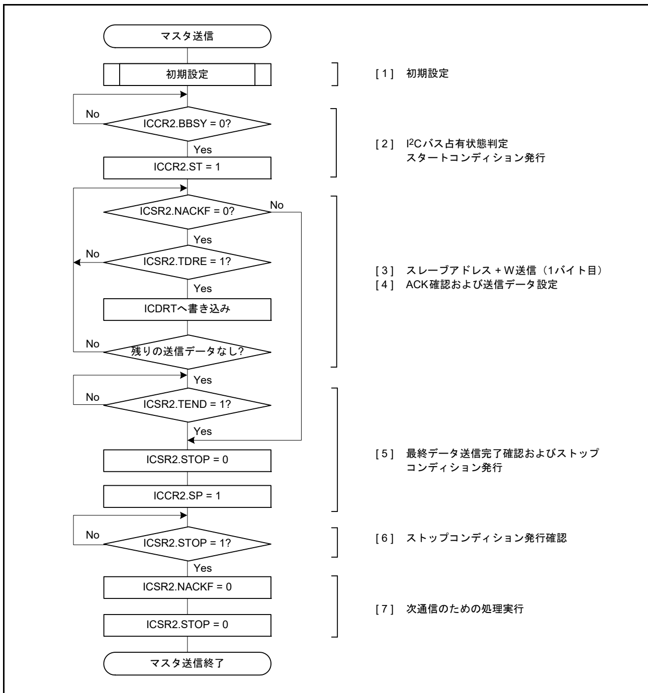
図 28.6 マスタ送信のフロー例
