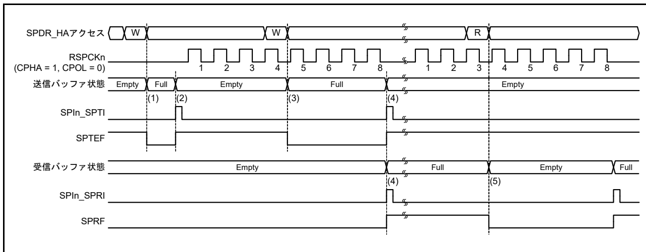
図 30.27 SPIn_SPTI、SPIn_SPRI 割り込みの動作例 (CPHA = 1、CPOL = 0)
