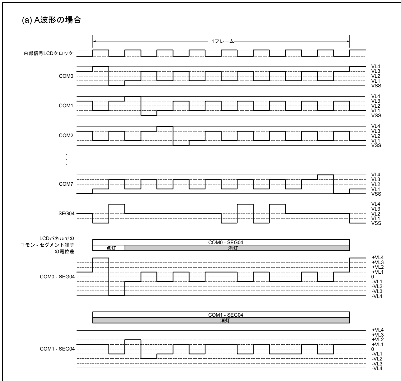
図 48.34 1/4 バイアス法を用いた SEG04 と各コモン信号との間の 4 時分割 LCD 駆動波形例 (1/2)
