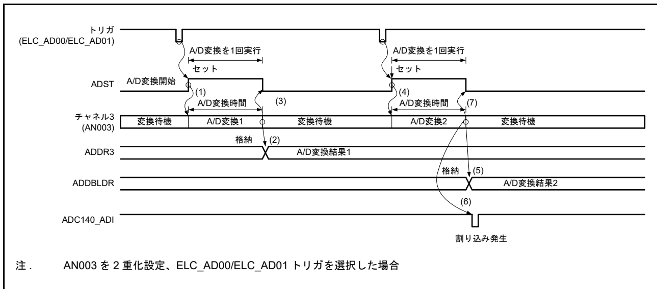
図 38.9 シングルスキャンモードの基本動作例 (ダブルトリガモード選択、AN003を2重化)
