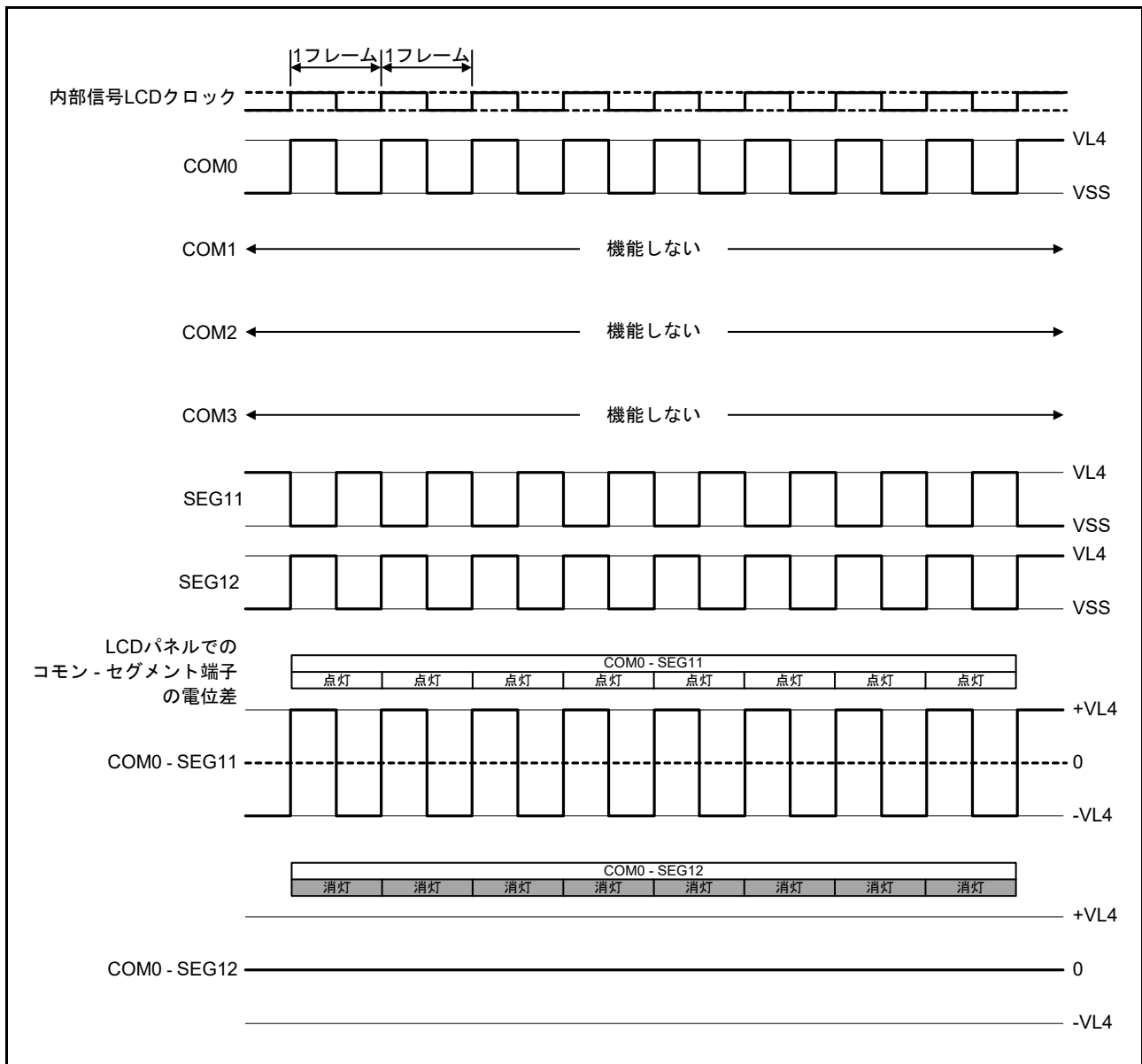
図 48.20 SEG11、SEG12、COM0 のスタティック LCD 駆動波形例
