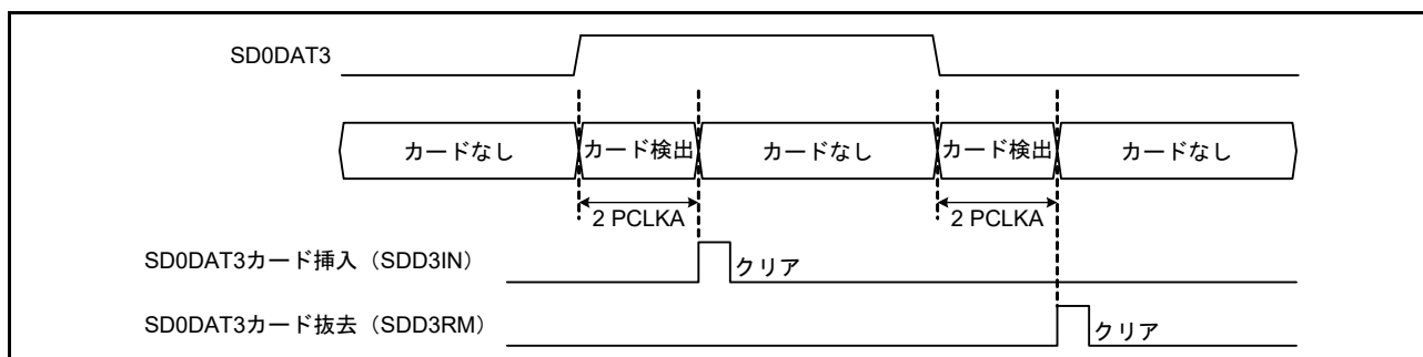
図 36.8 SD0DAT3 による SD カード検出
