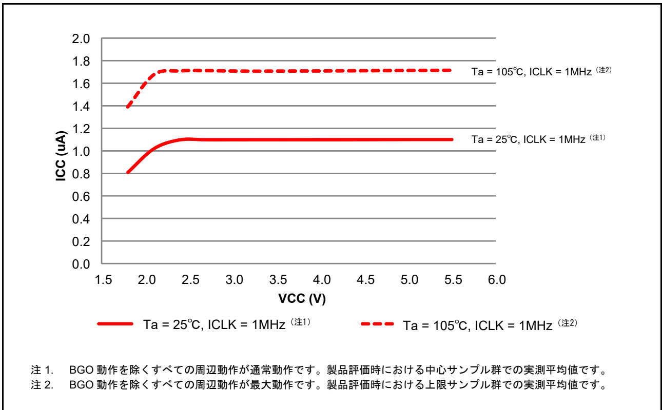
図 50.19 Low-speed モードにおける電圧依存性 (参考データ)
