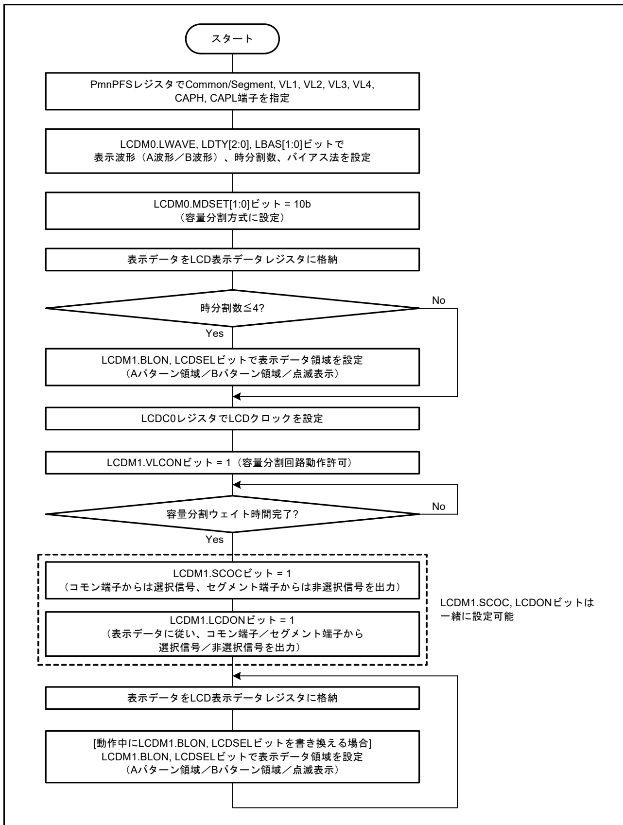
図 48.7 通常液晶波形表示での容量分割方式の設定手順
