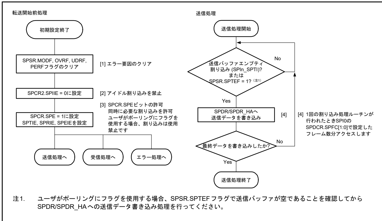
図 32.48 スレープモードでの送信フロー
