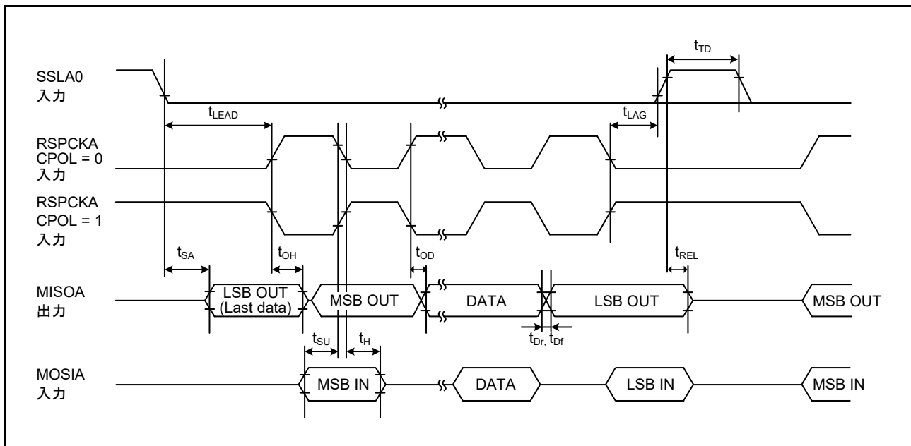
図 50.67 SPI タイミング (スレーブ、CPHA = 1)
