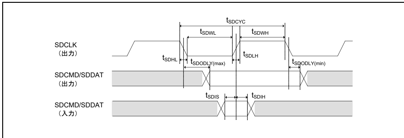
図 50.75 SD/MMC ホストインタフェース信号タイミング
