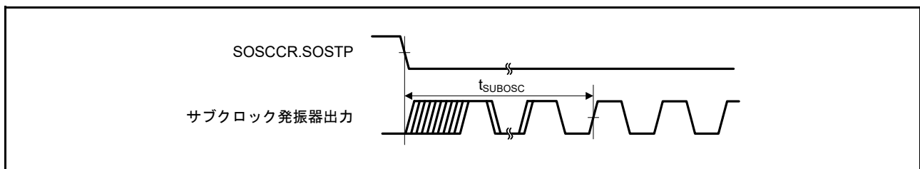
図 50.32 サブクロック発振開始タイミング
