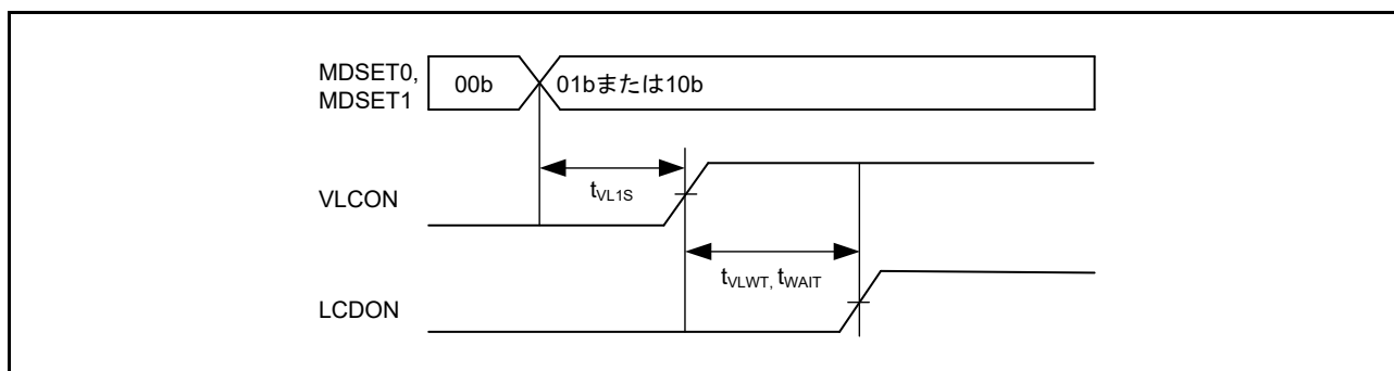
図 50.92 LCD 基準電圧セットアップ時間、昇圧待機時間、容量分割待機時間
