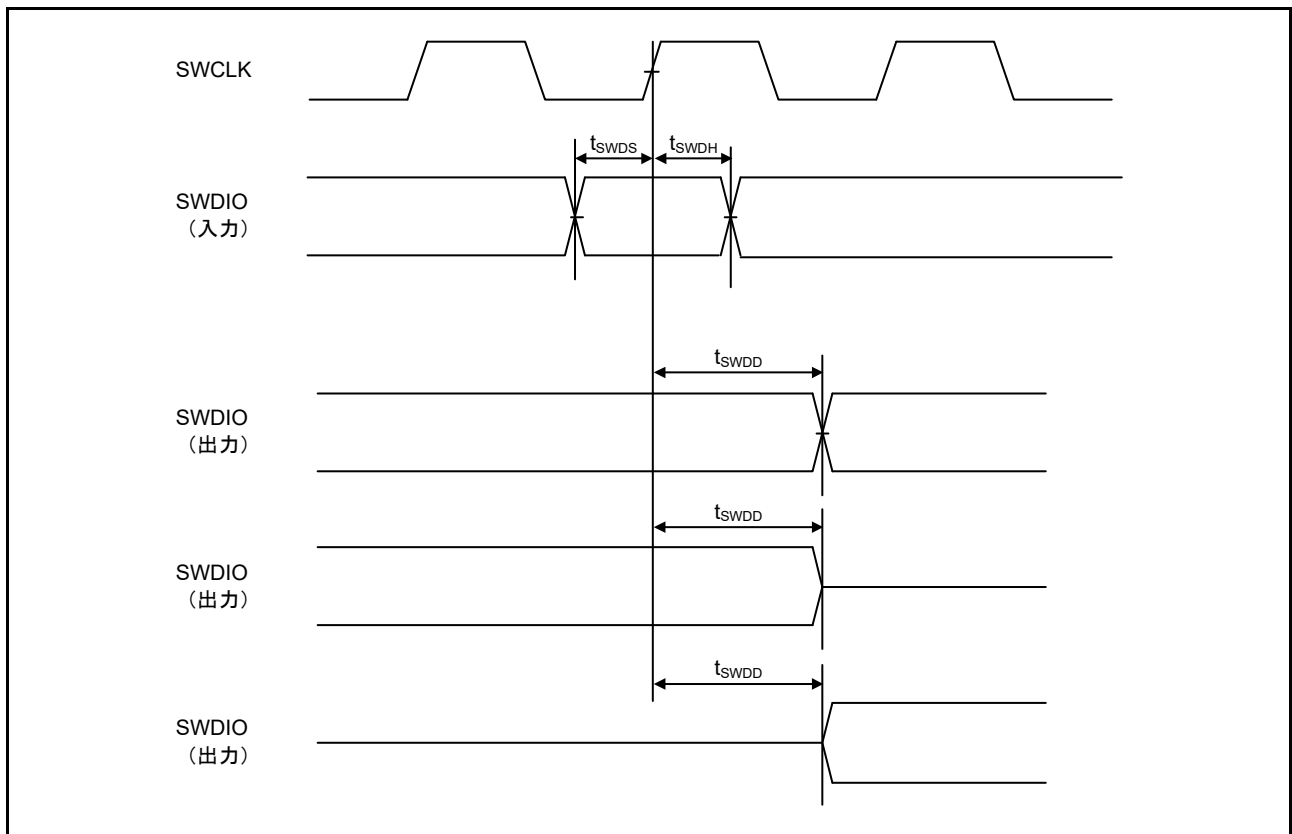
図 50.99 SWD 入出力タイミング
