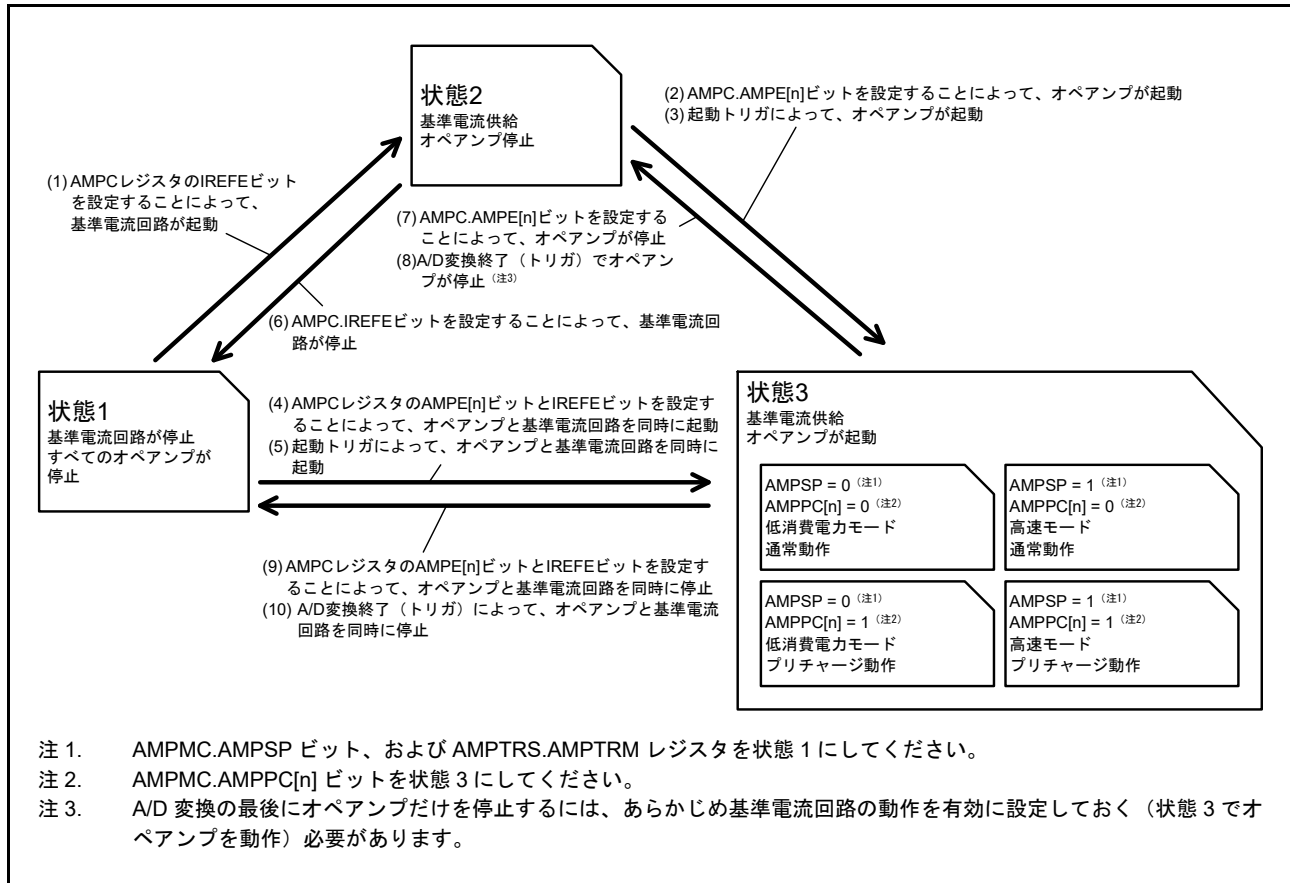
図 41.2 オペアンプの状態遷移
