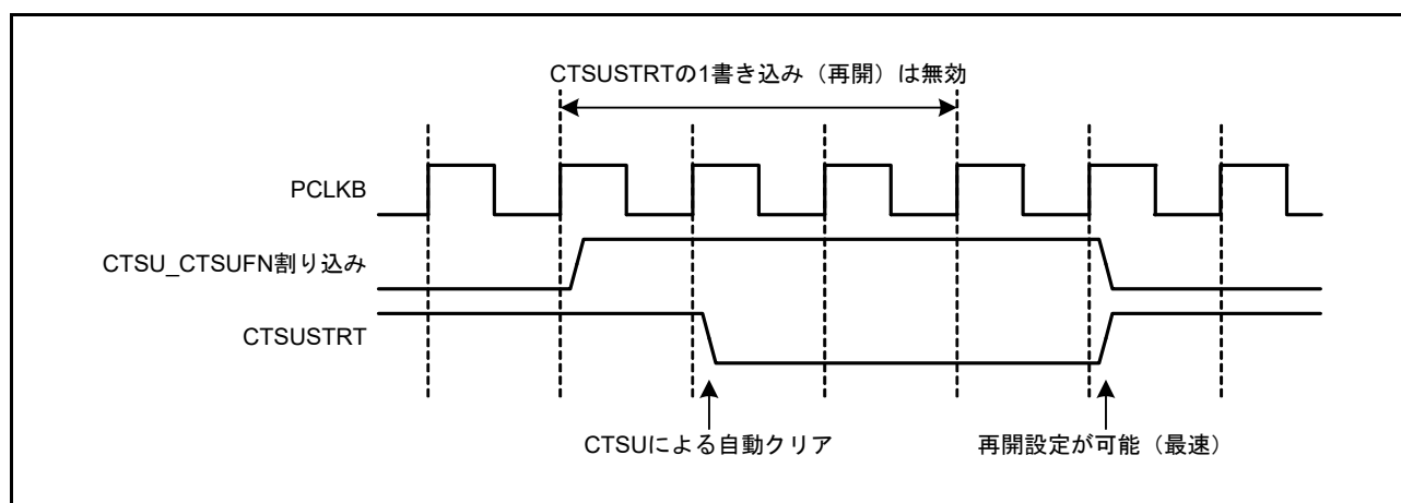
図 44.21 再開時の注意事項
