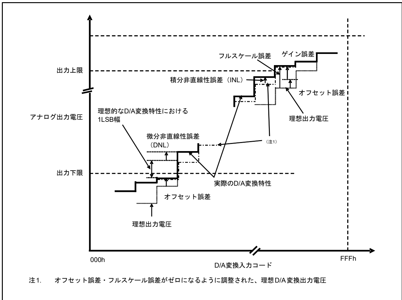
図 50.82 D/A コンバータ特性用語の解説図
