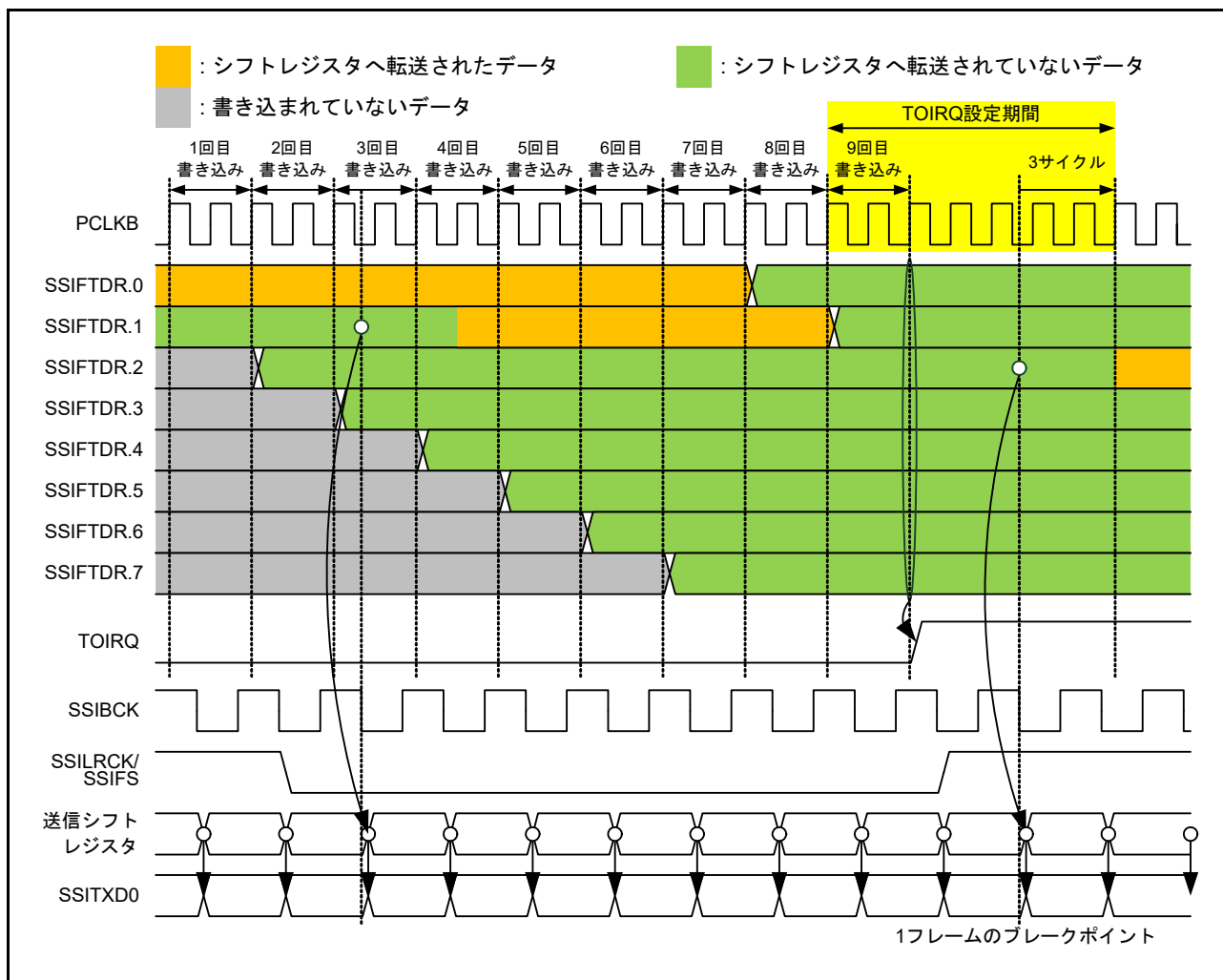
図 35.16 TOIRQ 設定タイミング
