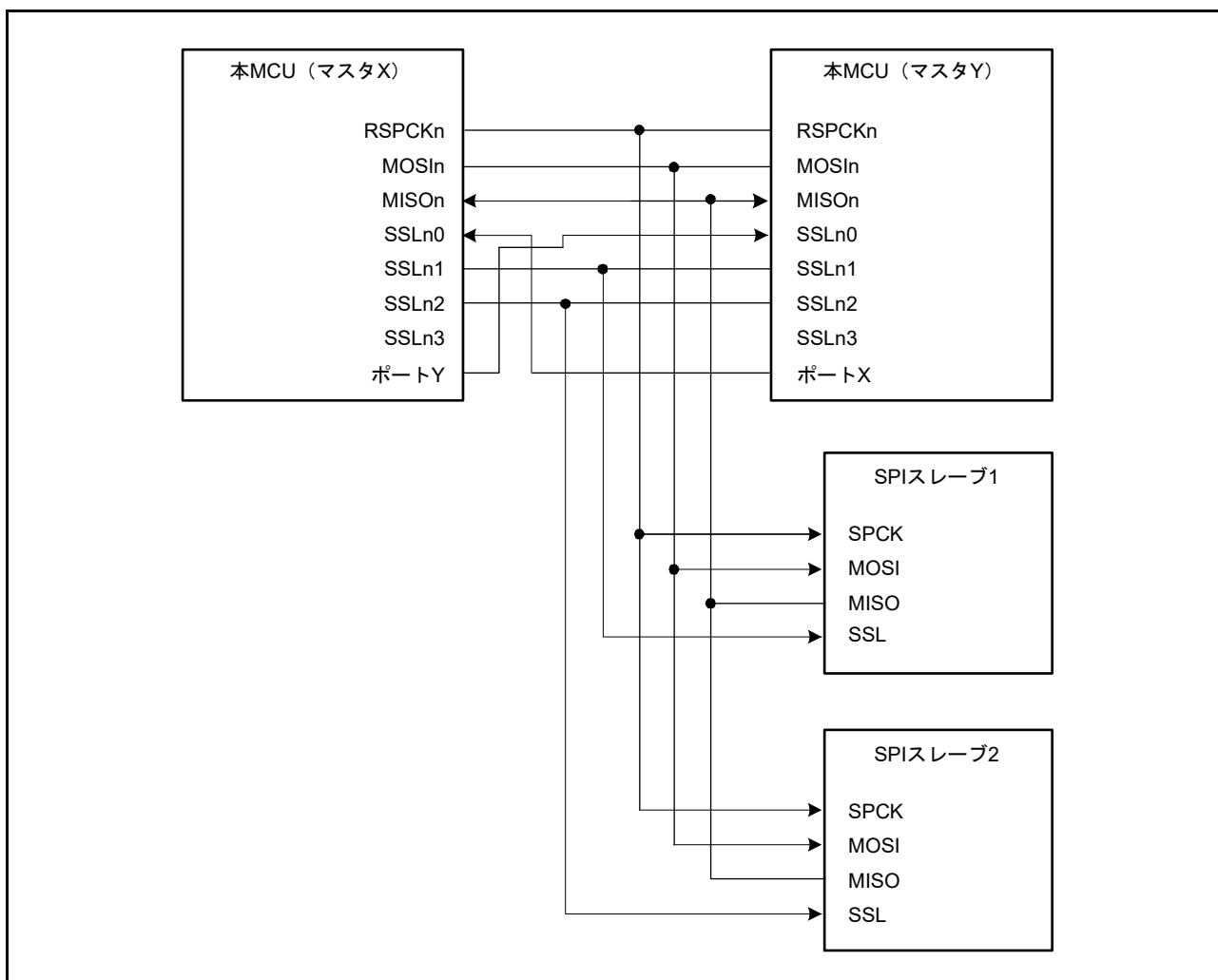
図 32.13 マルチマスタとマルチスレーブの構成例 (MCU はマスタ)
