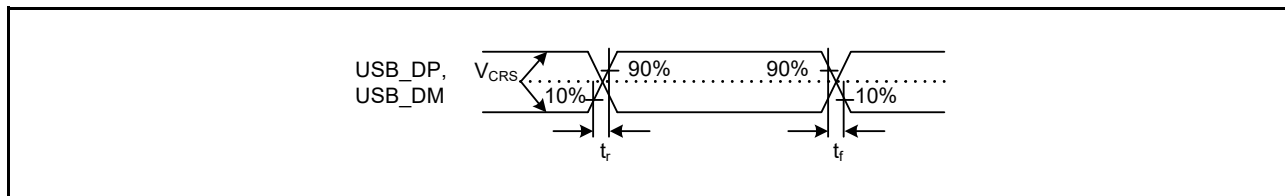
図 50.77 USB_DP および USB_DM 出力タイミング
