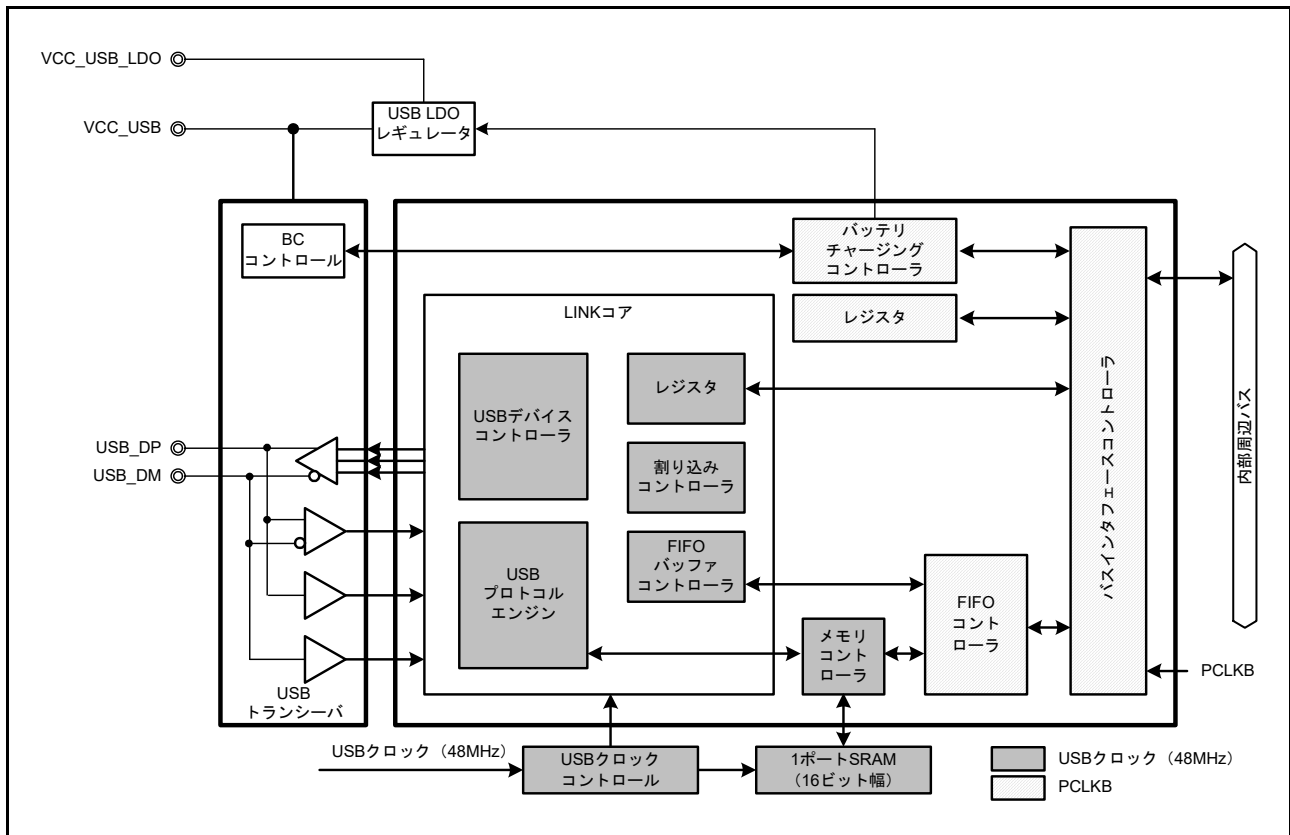
図 28.1 USBFS のブロック図
