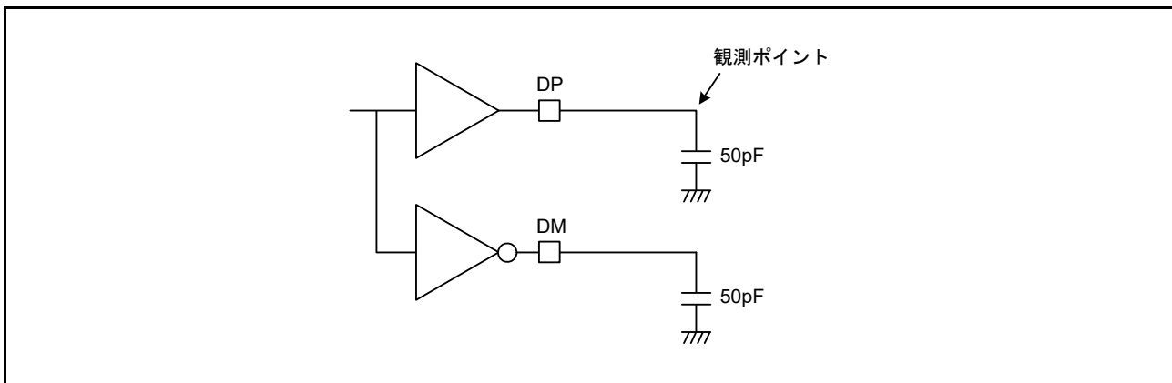
図 50.78 フルスピード (FS) 接続の測定回路
