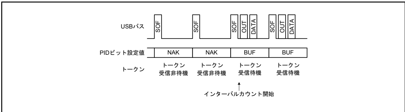
図 28.19 フレームとトークン受信待機の関係 (IITV = 0 の場合)
