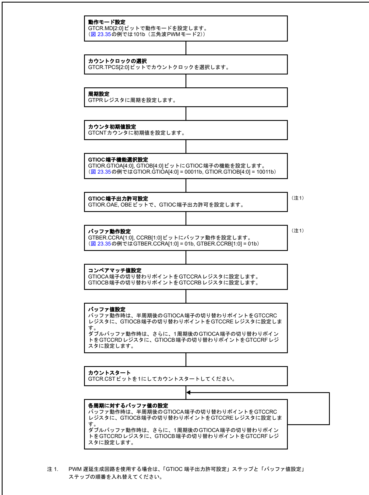
図 23.36 三角波 PWM モード 2 の設定例
