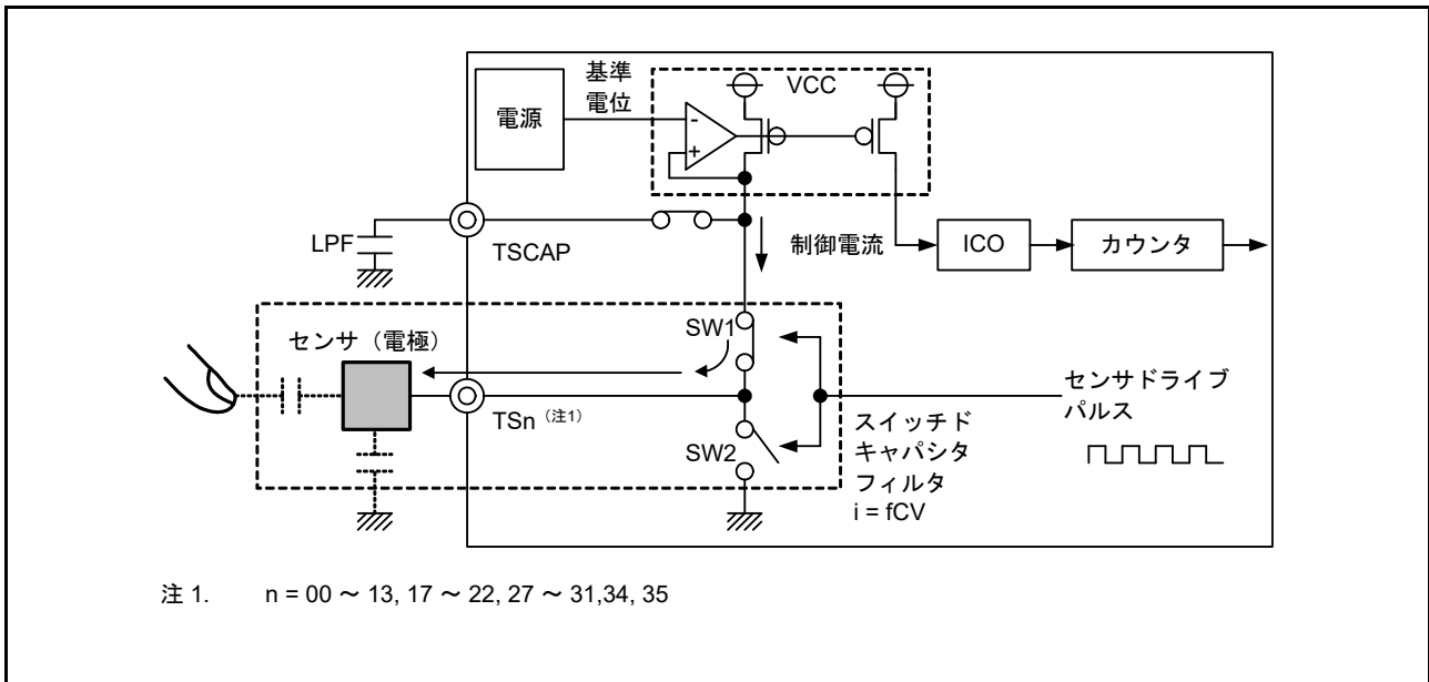
図 44.5 充電動作
