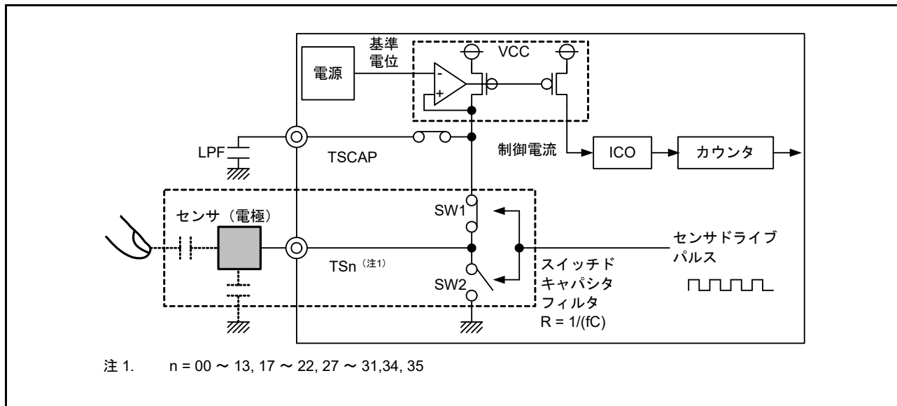
図 44.4 計測部回路
