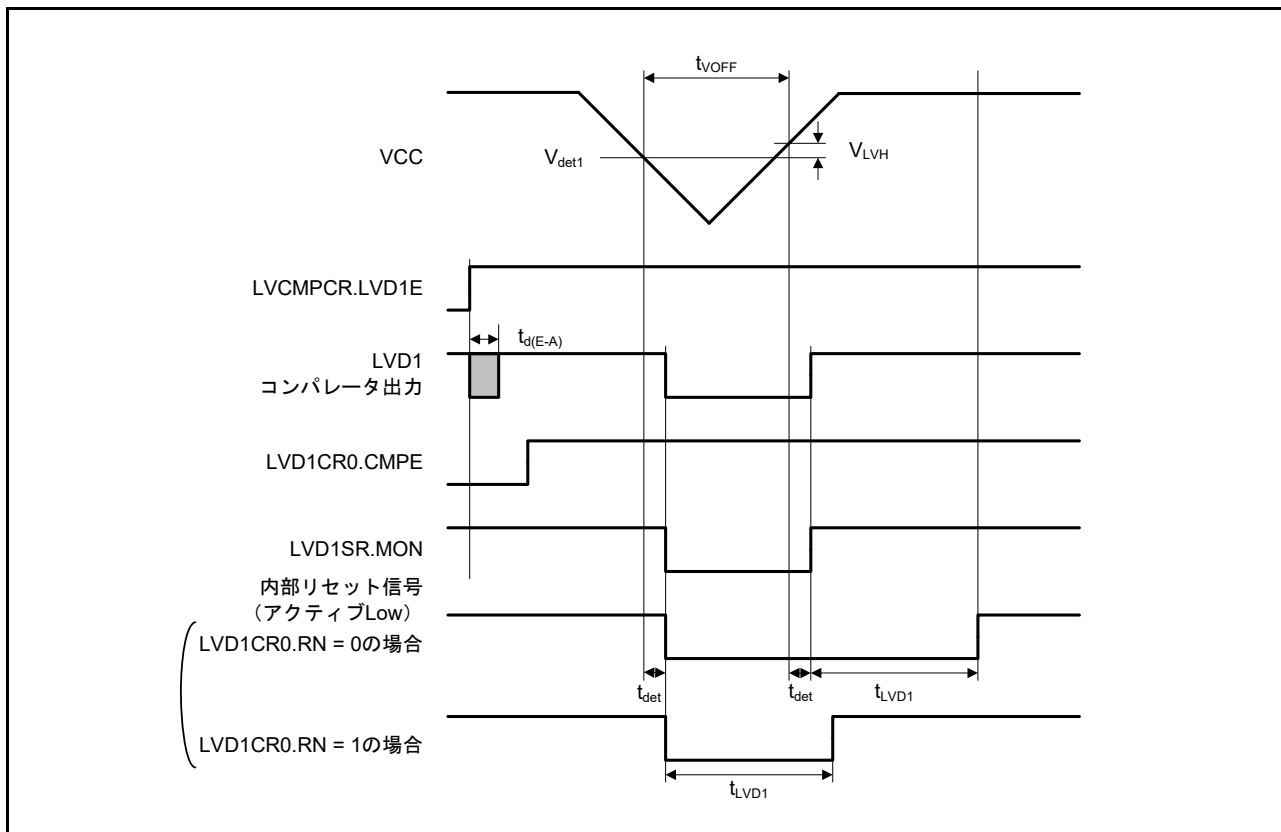
図 50.87 電圧検出回路タイミング ( V_{det1} )
