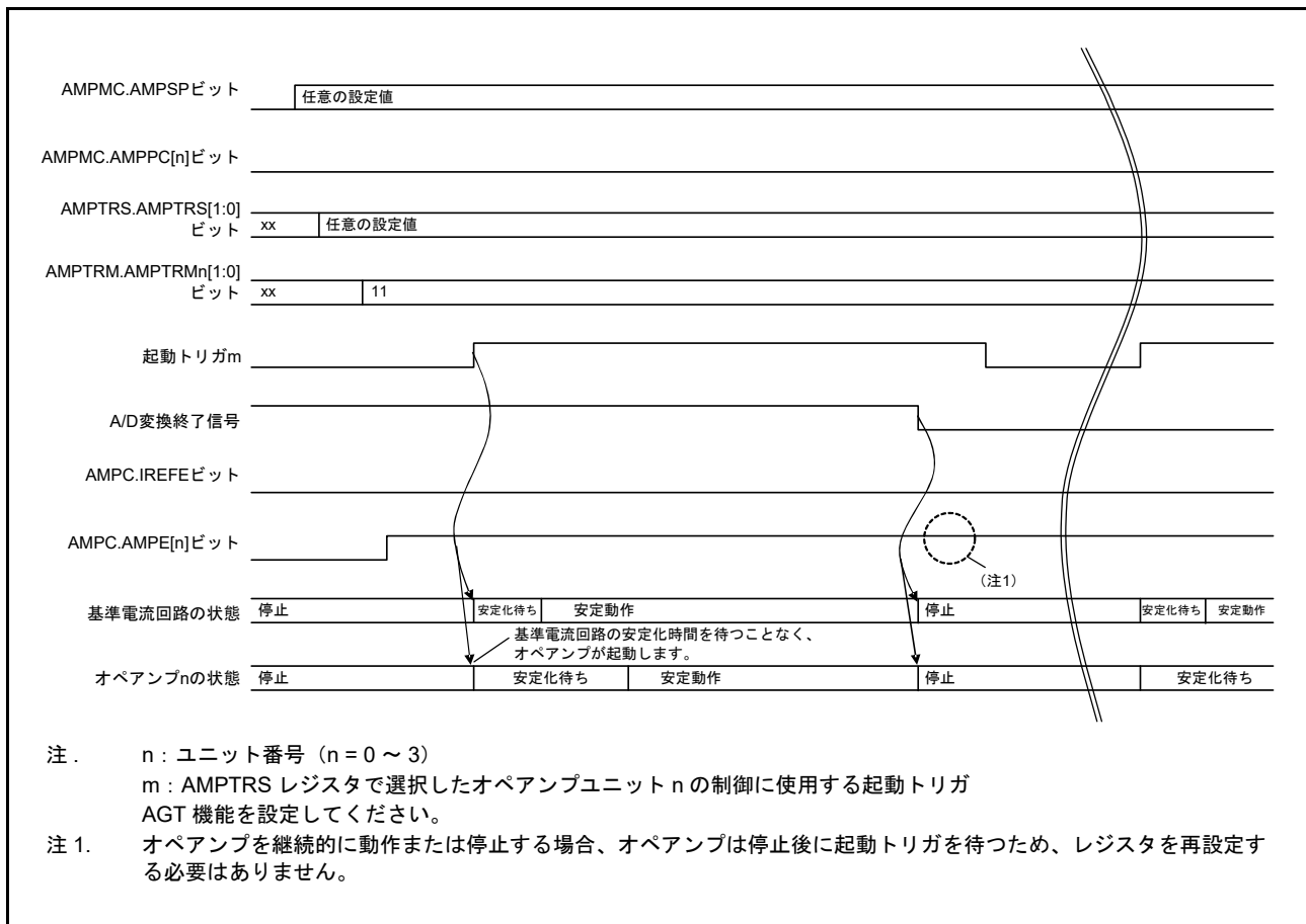
図 41.5 オペアンプの制御動作 (起動および A/D トリガモード (1)) (基準電流回路およびオペアンプを起動トリガによって起動し、A/D 変換終了 (トリガ) によって停止する場合)
