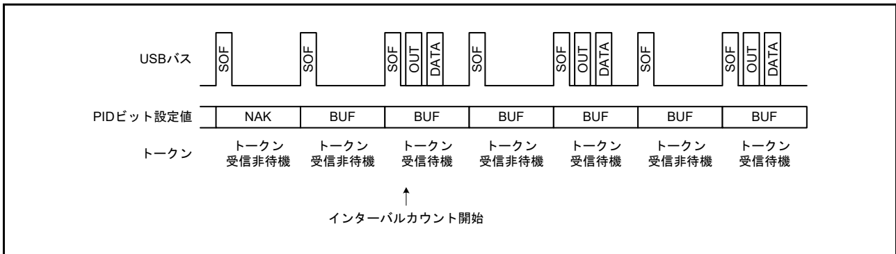
図 28.20 フレームとトークン受信待機の関係 (IITV ≠ 0 の場合)
