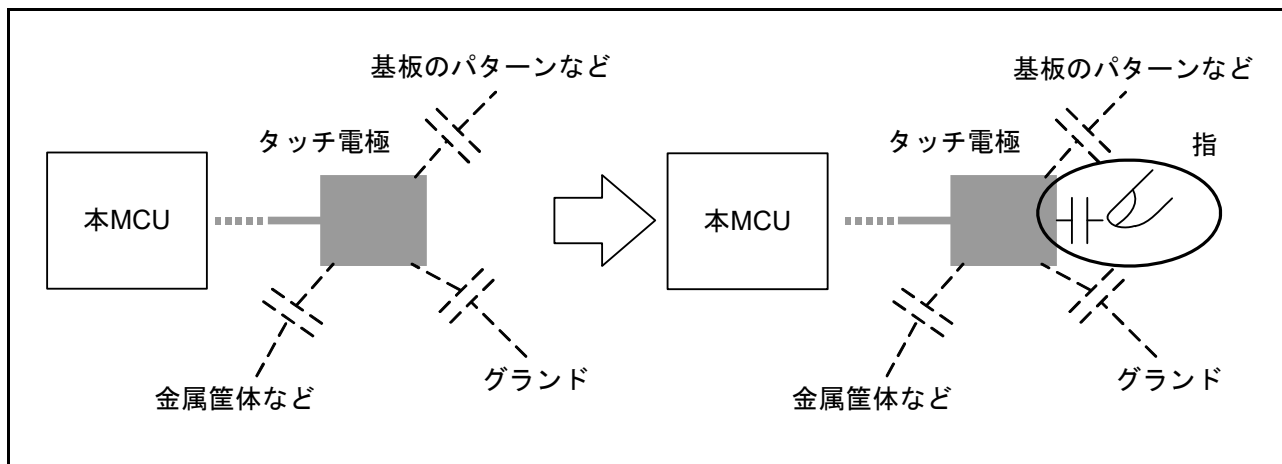
図 44.1 指による静電容量の増加
