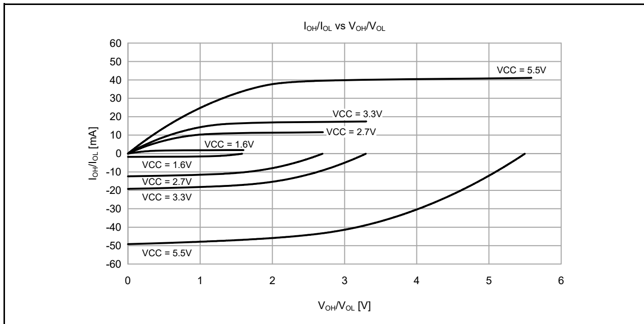
図 50.2 低駆動出力選択時の T_a = 25^\circ\text{C} での V_{OH}/V_{OL} および I_{OH}/I_{OL} 電圧特性 (参考データ)
