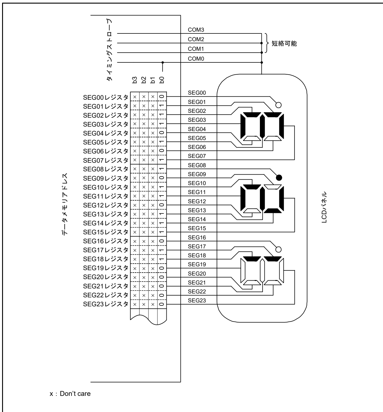
図 48.19 スタティック LCD パネルの接続例
