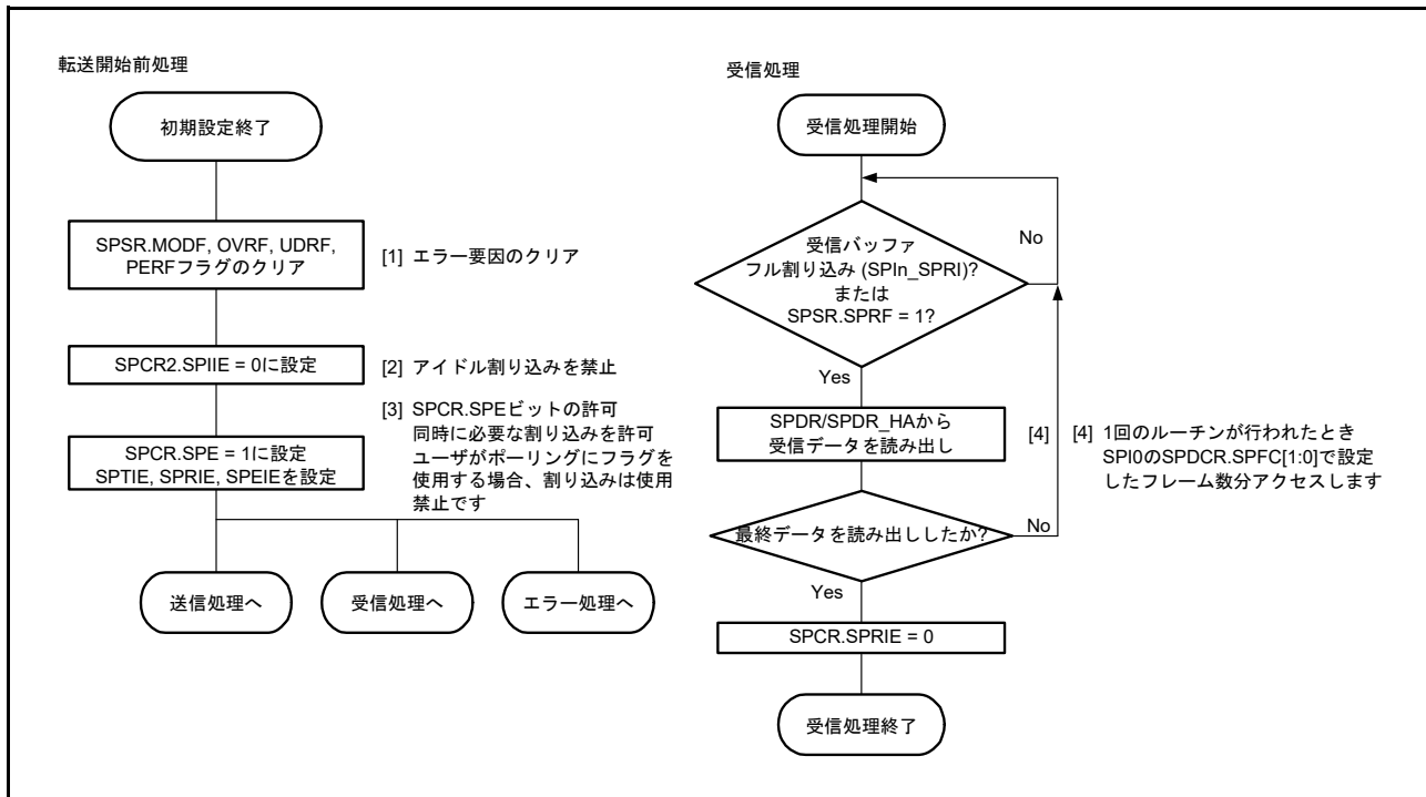
図 32.49 スレープモードでの受信フロー
