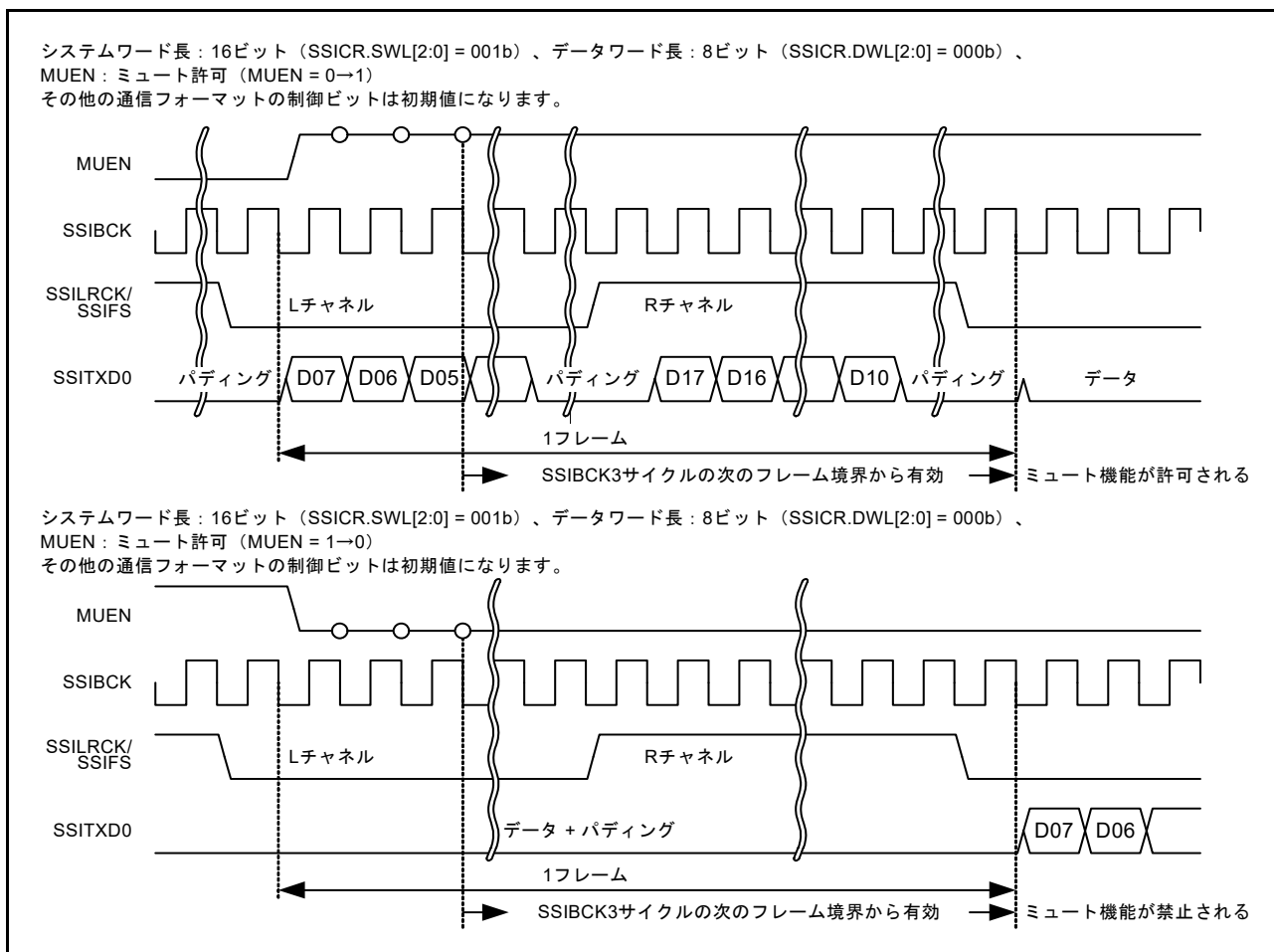
図 35.4 ミュート機能設定時の送信データ
