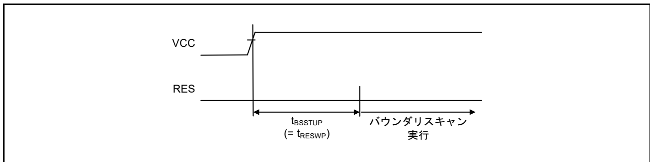
図 50.95 バウンダリスキャン回路起動タイミング
