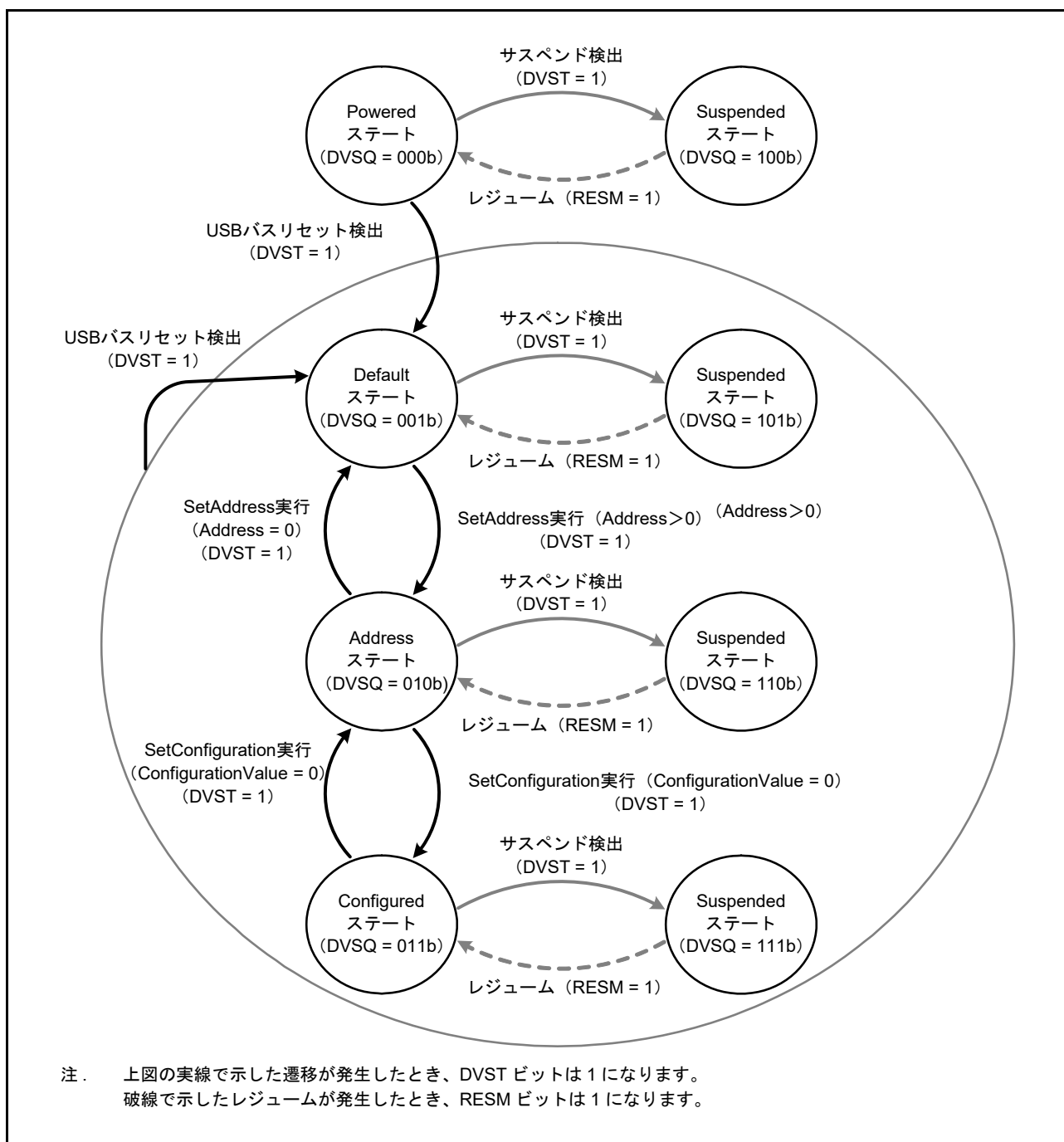
図 28.15 デバイスステートの遷移
