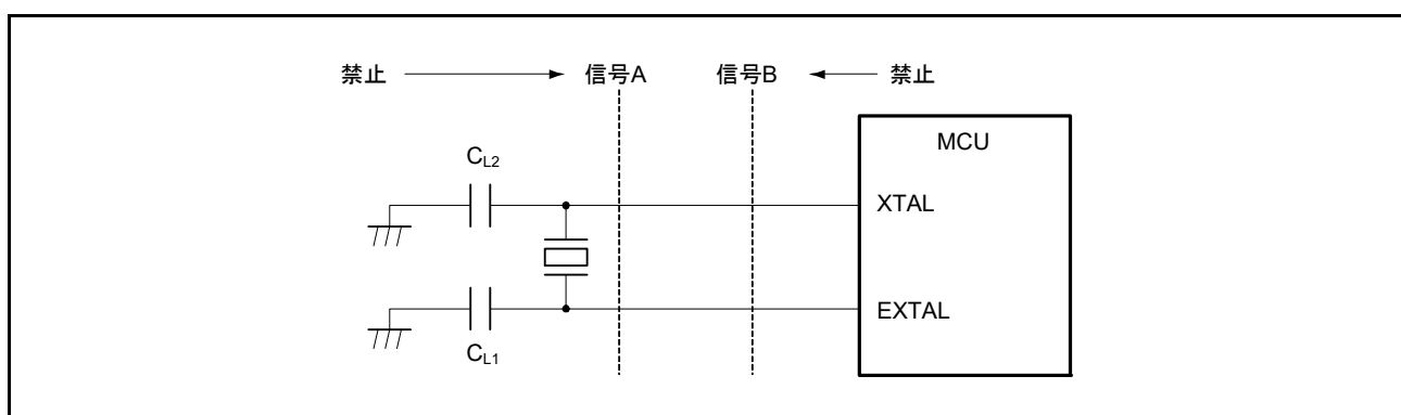
図 9.8 発振回路部のボード設計での信号ルーティング (メインクロック発振器の場合、サブクロック発振器も同様)
