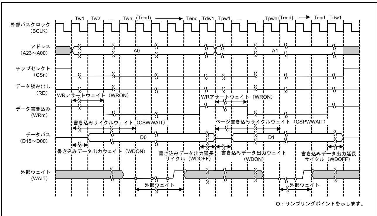
図 15.28 バイトストローブモード時の 16 ビットバス空間に対するページライトアクセスの外部ウェイトタイミング例 (EBCLK 端子出力選択ビットで BCLK の 1 分周を選択した場合) (n = 0 ~ 3, m = 0, 1)
