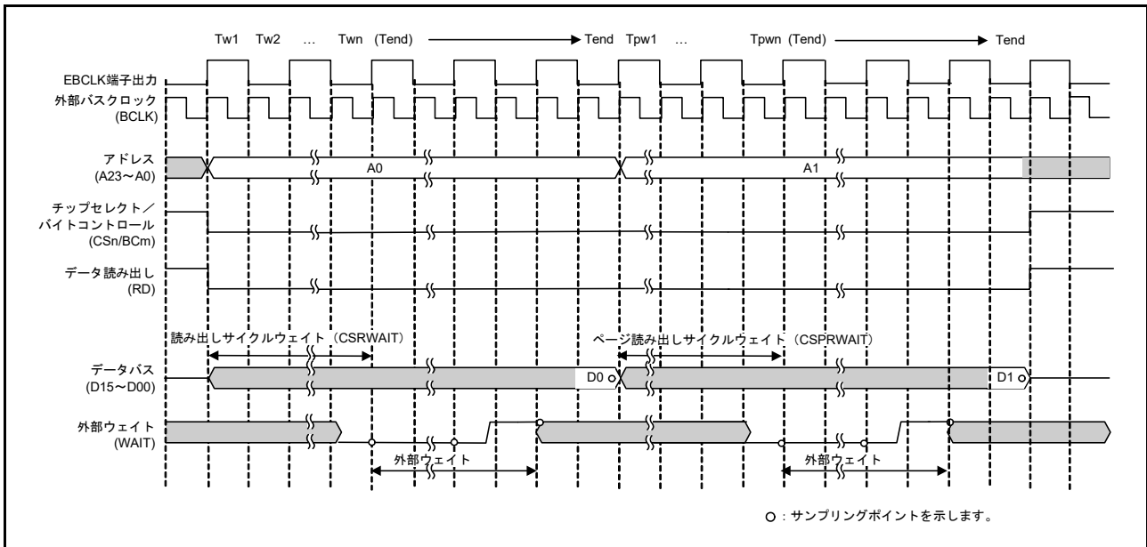
図 15.27 16 ビットバス空間に対するページリードアクセスの外部ウェイトタイミング例 (EBCLK 端子出力選択ビットで BCLK の 2 分周を選択した場合) (n = 0 ~ 3, m = 0, 1)
