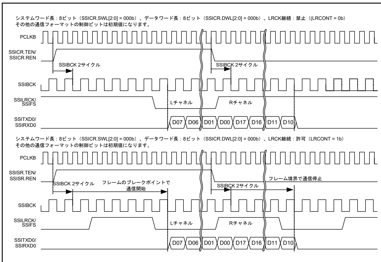
図 35.31 LR クロック/フレーム同期継続の動作例
