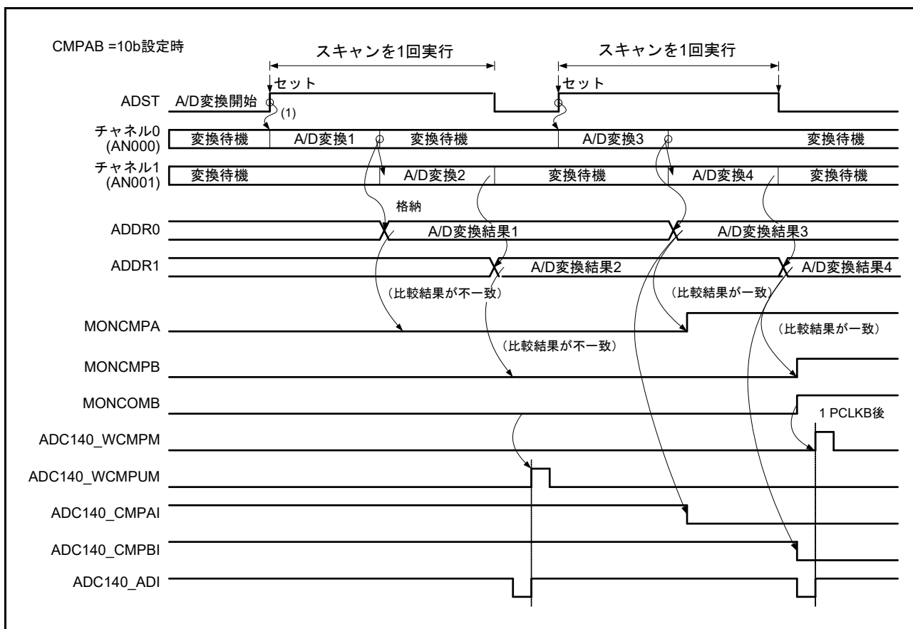
図 38.23 コンペア機能のイベント出力動作例 (AN000 ~ AN003 を比較)
