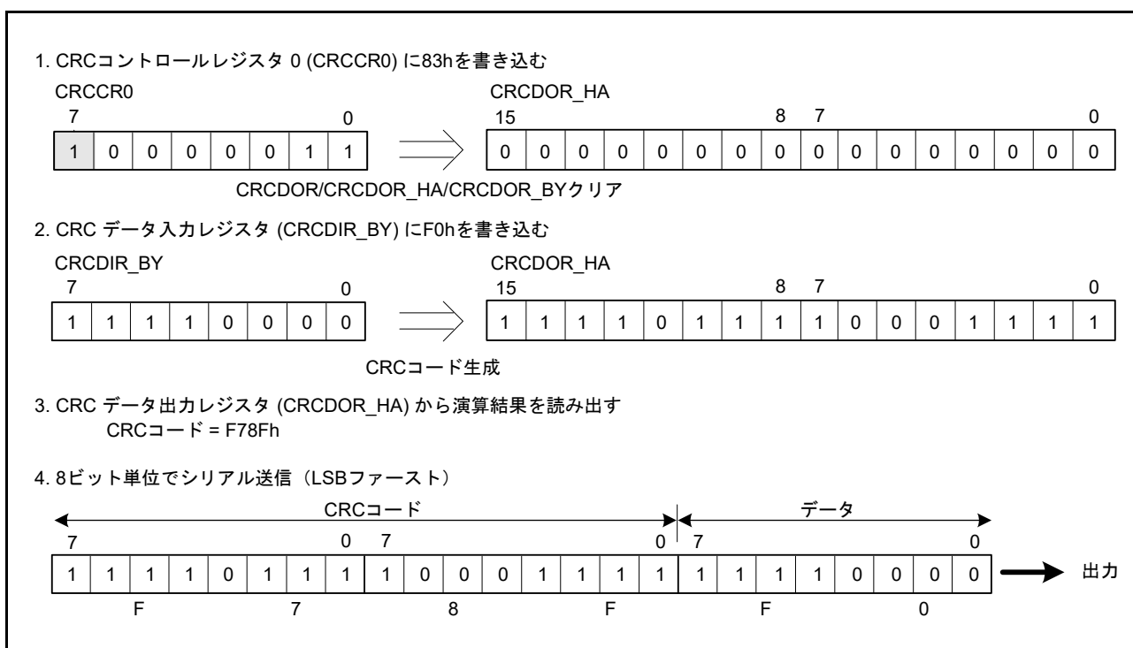
図 34.2 LSB ファーストのデータ送信
