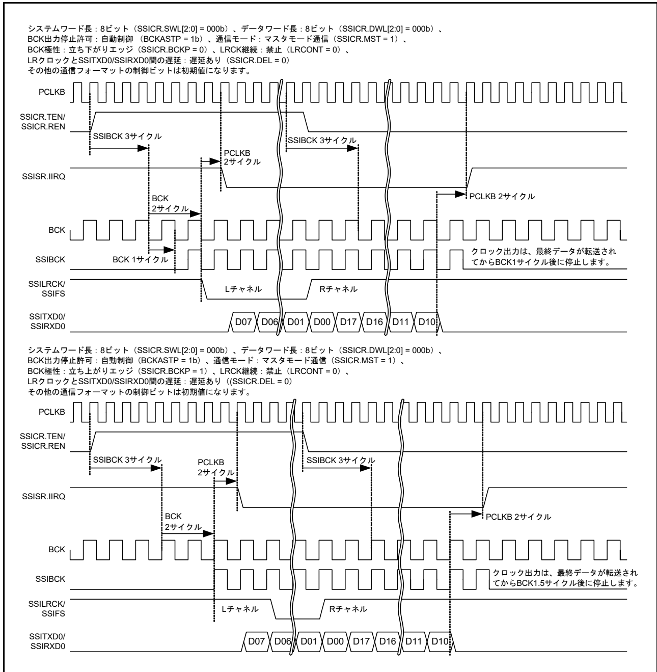
図 35.33 BCKASTP ビットの動作例 (BCKASTP = 1 での通信の場合)
