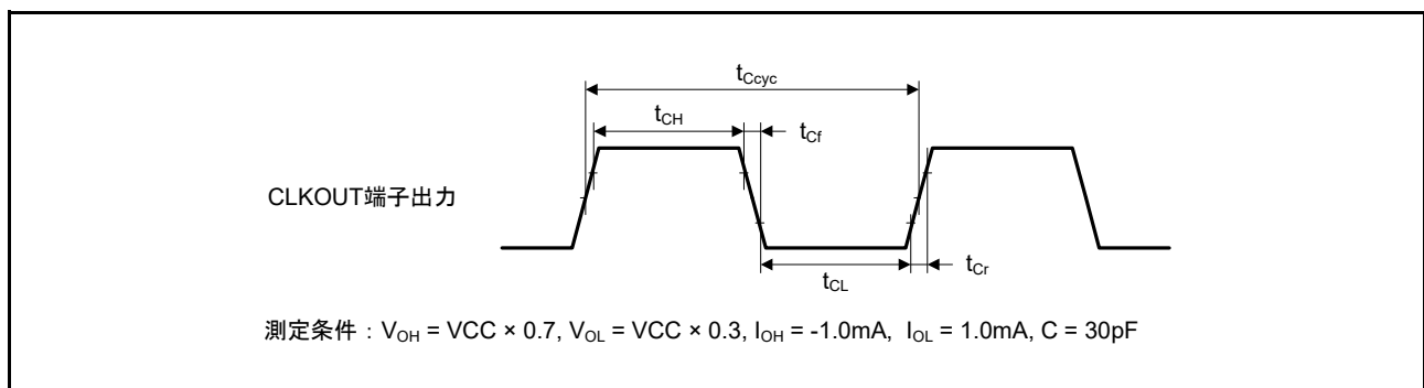
図 50.76 CLKOUT 出力タイミング
