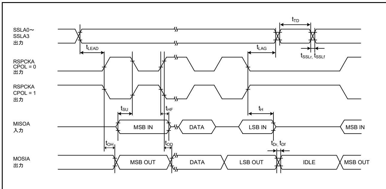
図 50.65 SPI タイミング (マスタ、CPHA = 1) (ビットレート : PCLKA を 2 分周に設定)
