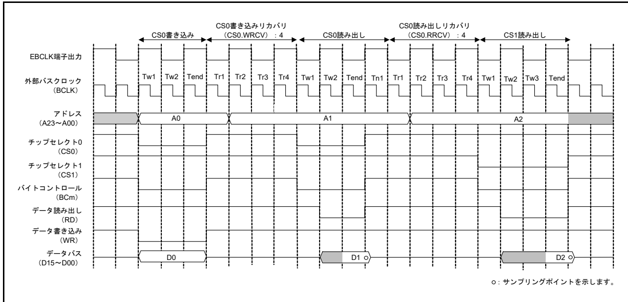
図 15.34 EBCLK 端子出力選択ビットで BCLK の 2 分周を設定した場合のリカバリサイクルの動作例 (セパレートバスインタフェースによるノーマルアクセスの場合) (m = 0, 1)
