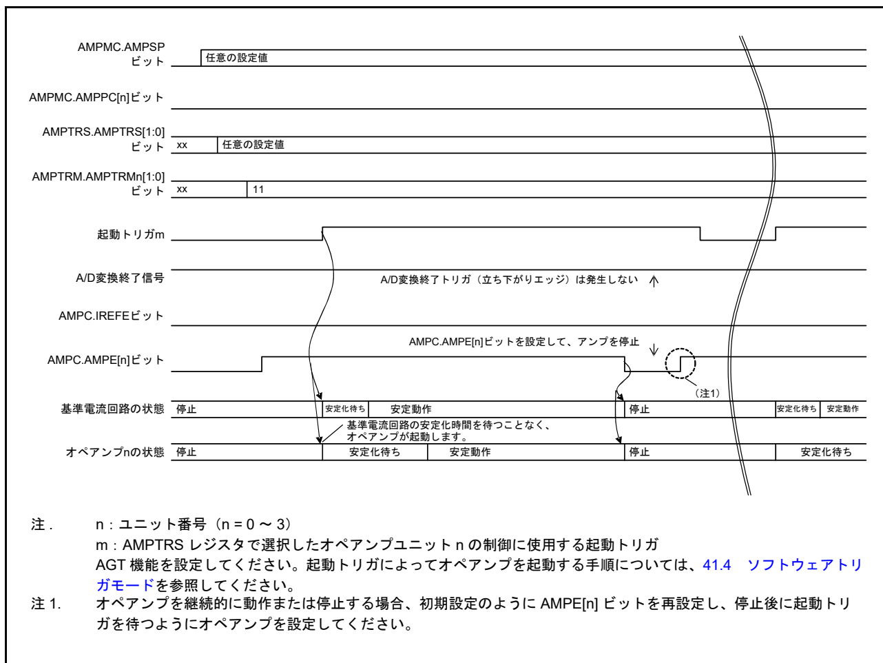
図 41.6 オペアンプの制御動作 (起動および A/D トリガモード (2)) (基準電流回路およびオペアンプを起動トリガによって起動し、AMPC レジスタの設定によって基準電流回路およびオペアンプを停止する場合)
