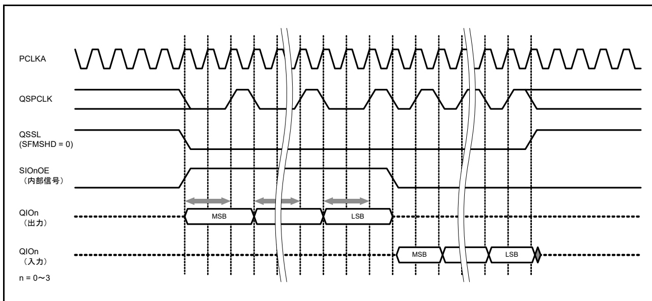
図 33.13 SFMOSW ビットを使用したシリアルデータ出力のセットアップ時間調整
