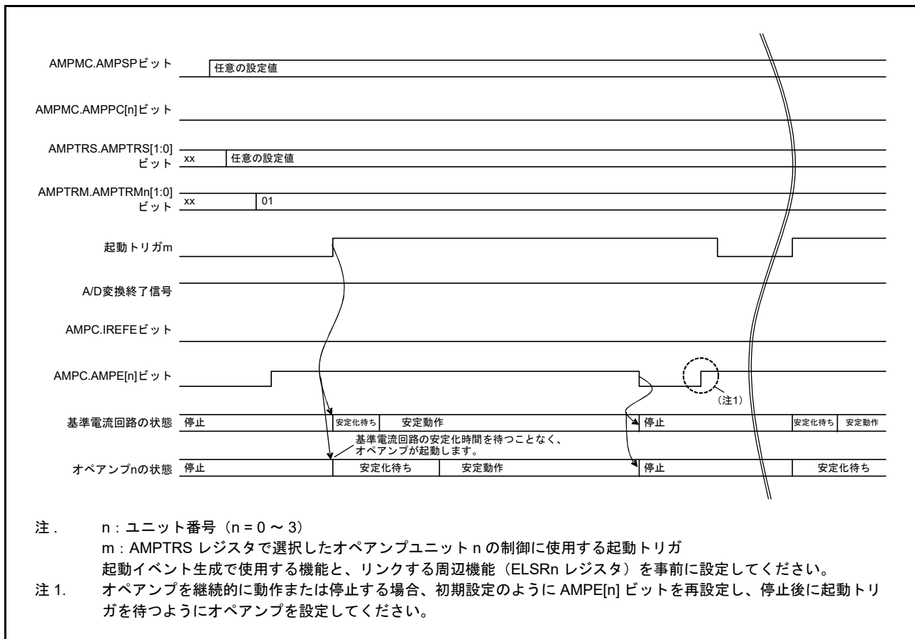
図 41.4 オペアンプの制御動作 (起動トリガモードによる起動) (基準電流回路およびオペアンプを起動トリガによって起動し、AMPC レジスタ設定によって停止する場合)
