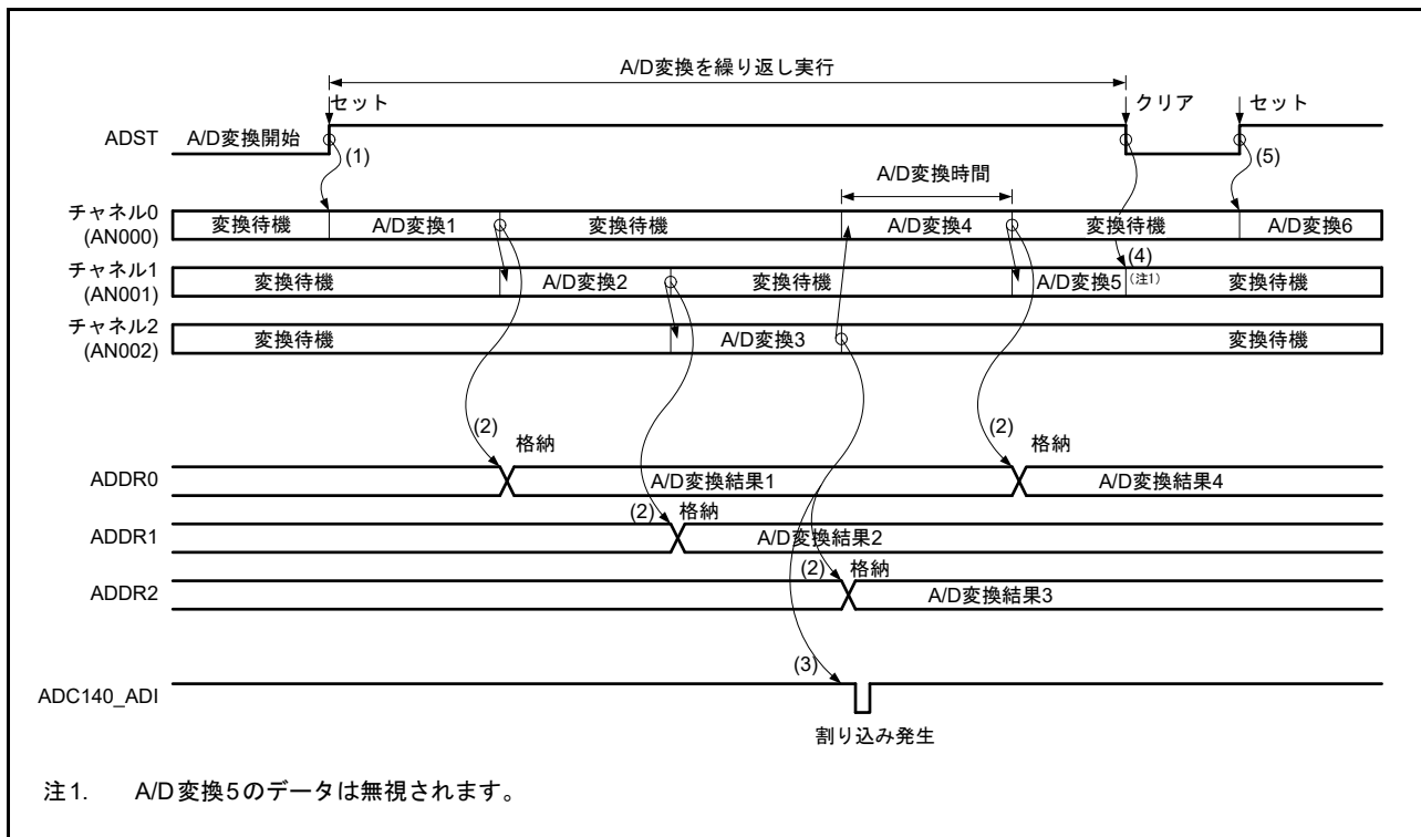
図 38.11 連続スキャンモードの基本動作例 (AN000 ~ AN002 選択)
