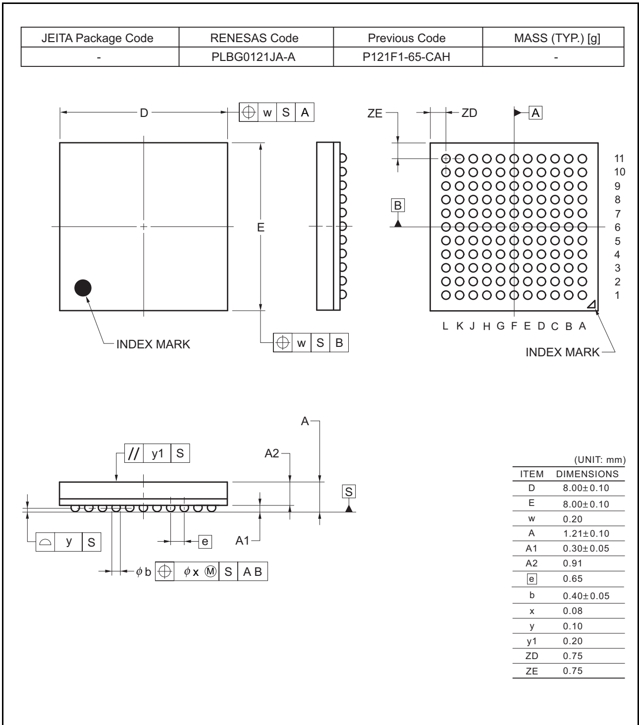
図 2.3 121-pin BGA
