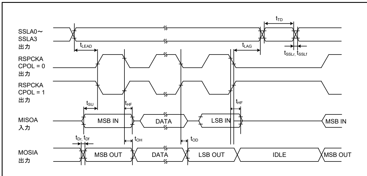
図 50.63 SPI タイミング (マスタ、CPHA = 0) (ビットレート : PCLKA を 2 分周に設定)
