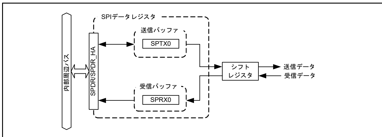
図 32.3 SPDR/SPDR_HA レジスタの構成図 (SPI1 の場合)
