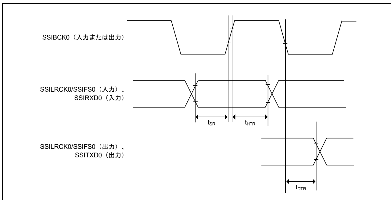
図 50.72 SSIE データ送受信タイミング (SSICR.BCKP = 0)
