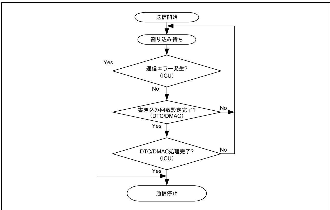
図 35.50 送信手順
