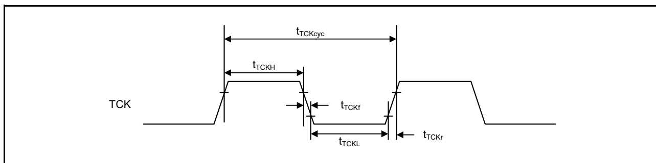
図 50.96 JTAG TCK タイミング
