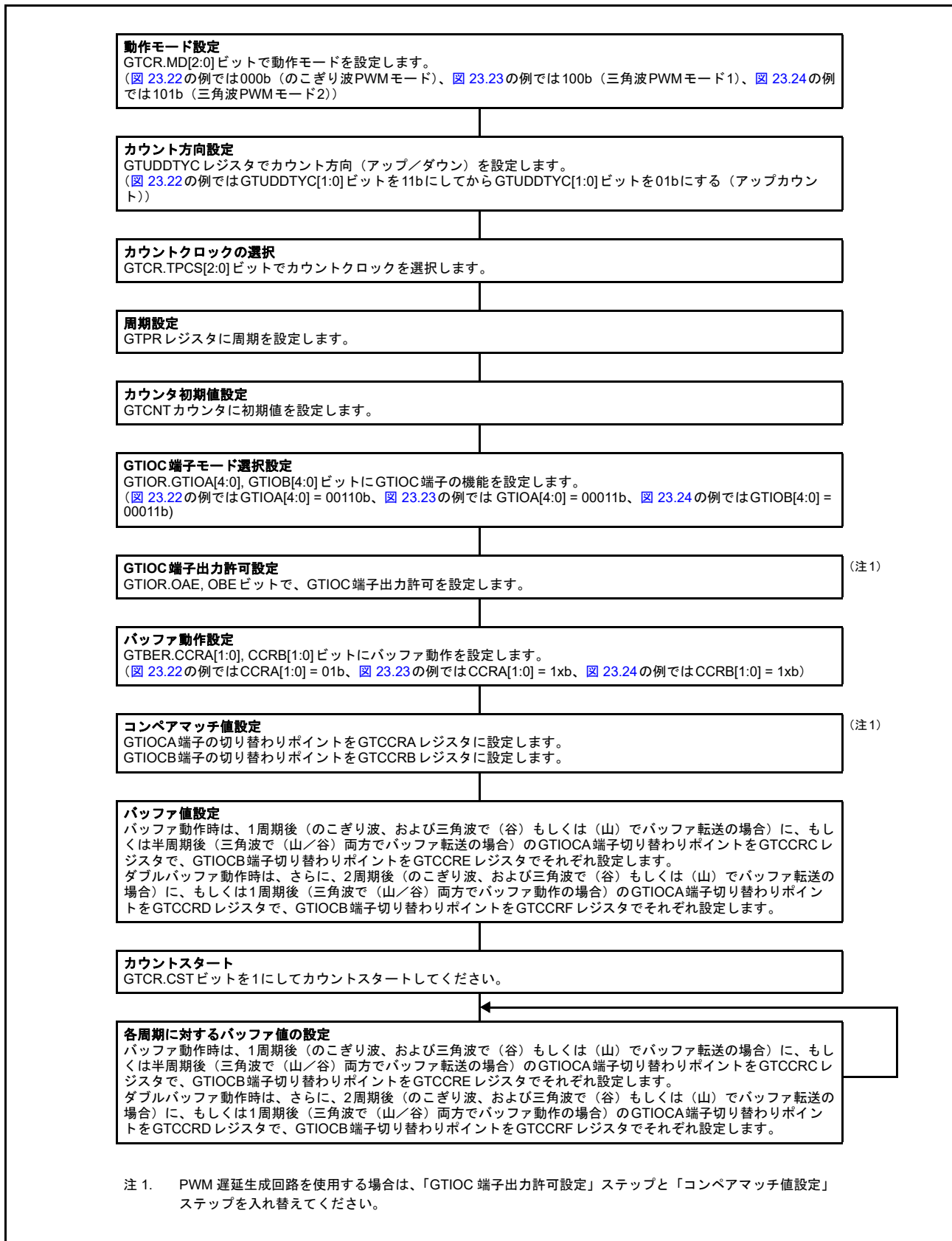
図 23.25 GTCCRA、GTCCRB レジスタのバッファ動作の設定例 (アウトプットコンペア時)
