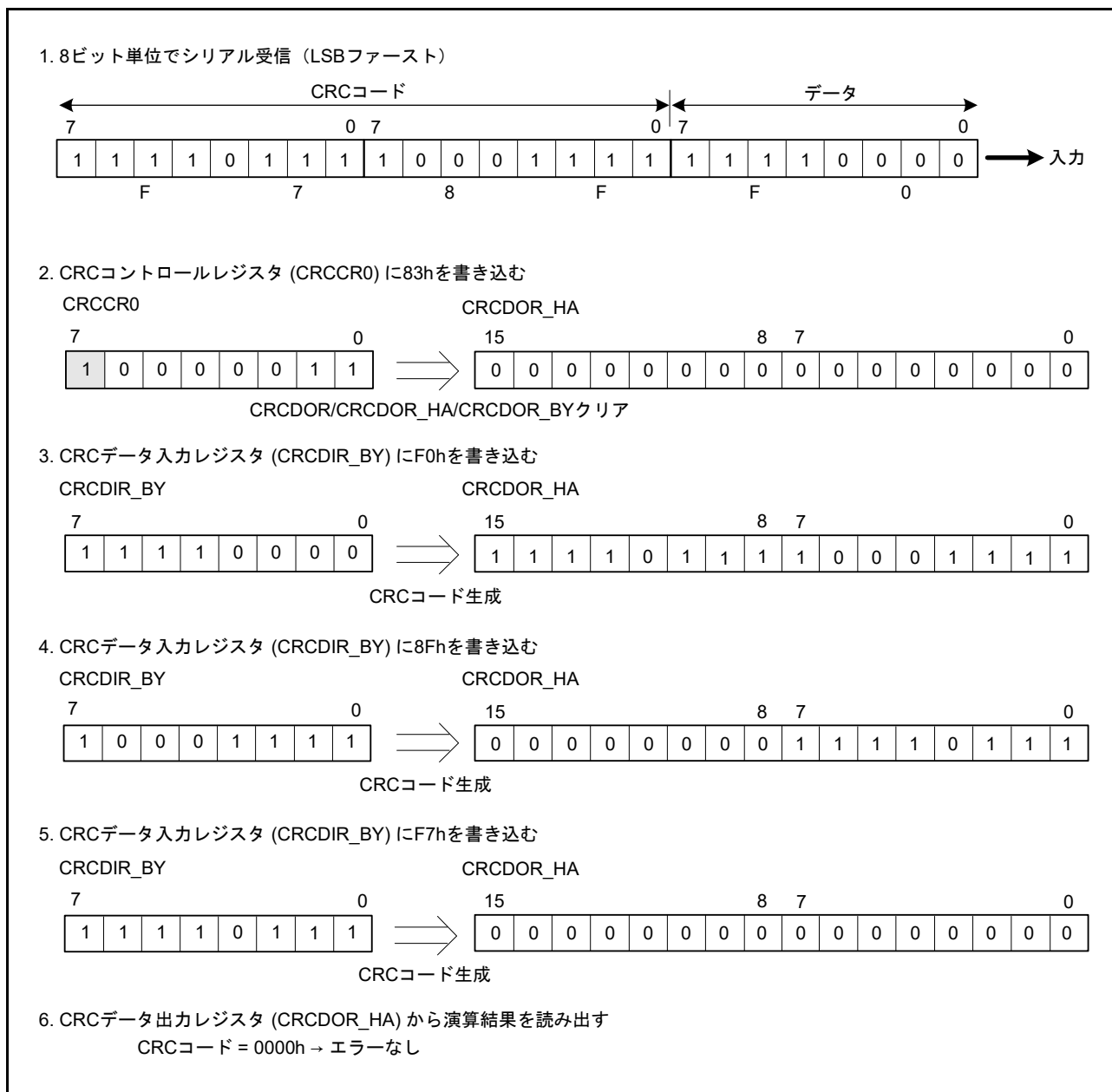
図 34.4 LSB ファーストのデータ受信
