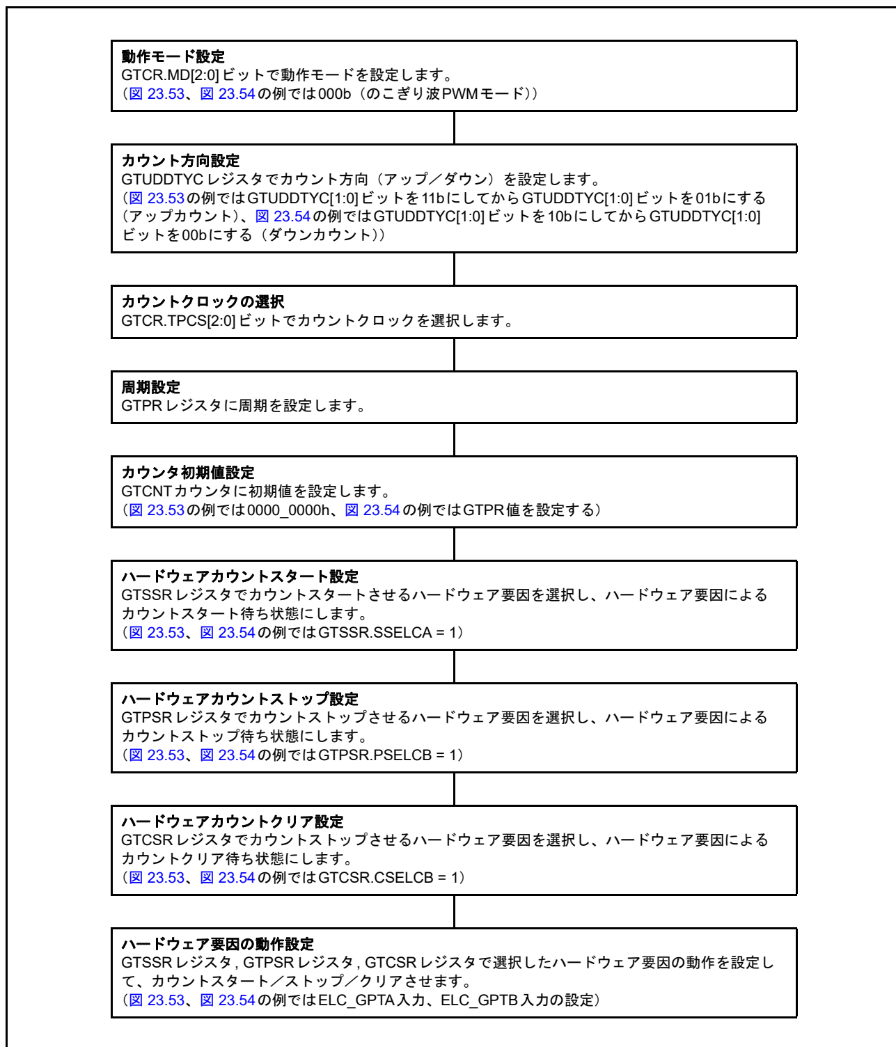
図 23.55 ハードウェア要因によるカウンタクリア動作設定例
