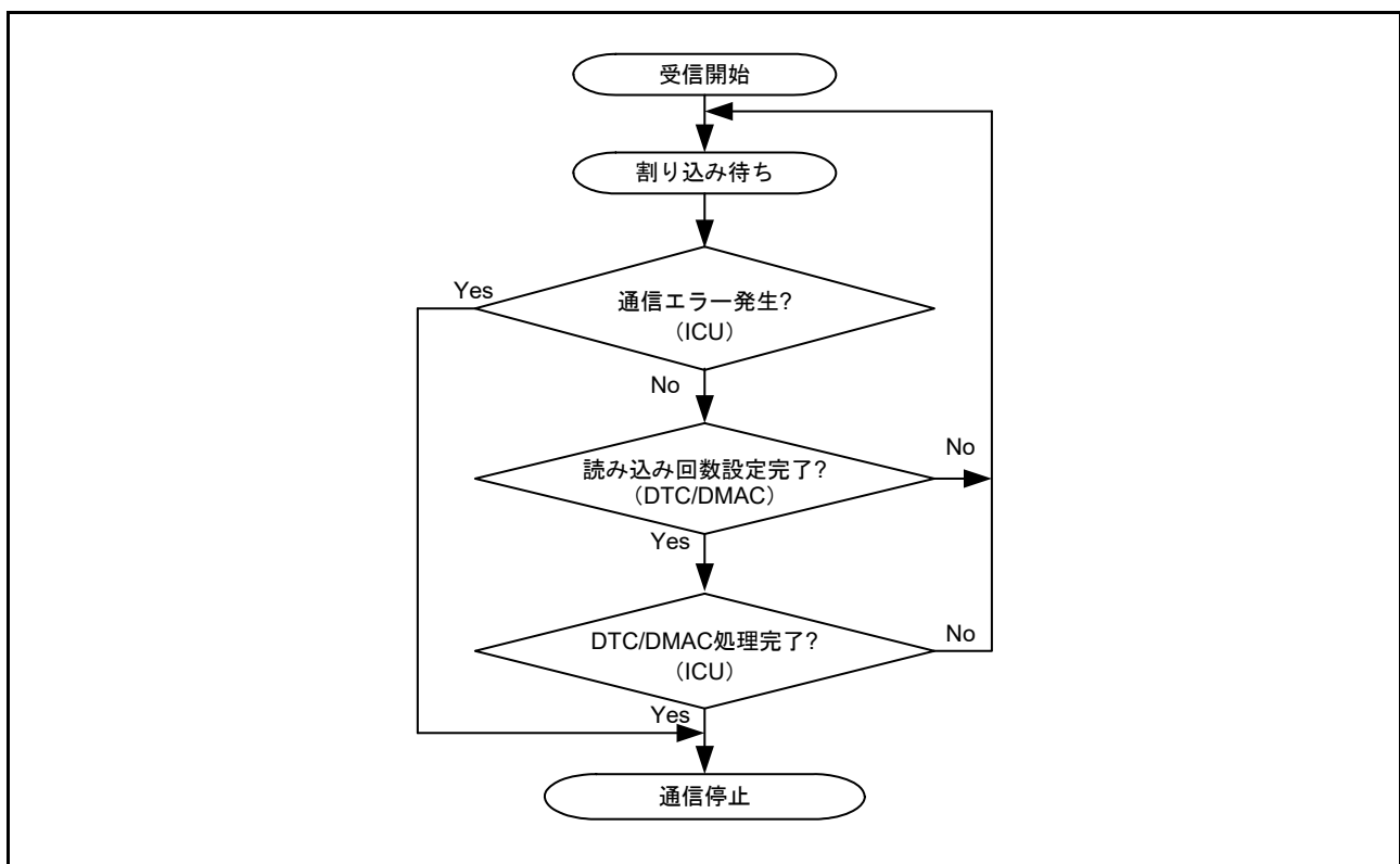
図 35.51 受信手順
