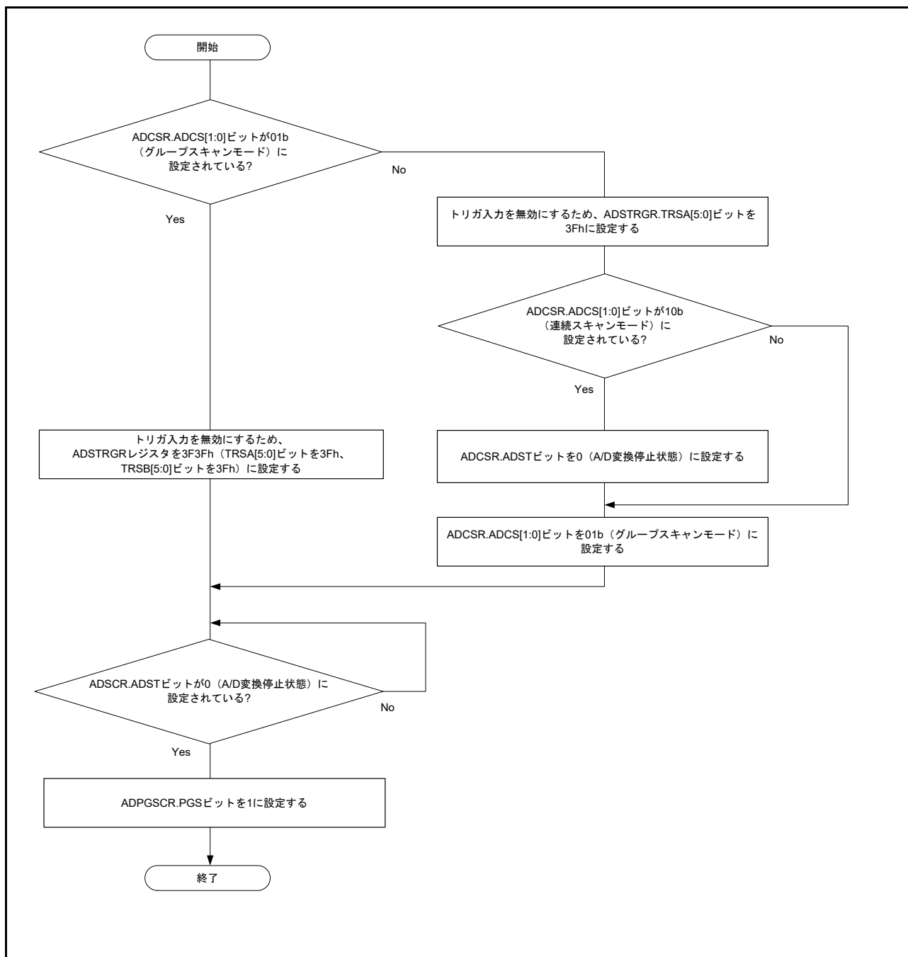
図 38.15 ADPGSCR.PGS ビット設定時のフロー
