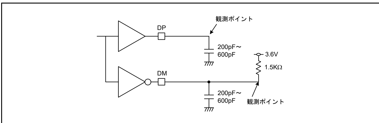
図 50.79 ロースピード (LS) 接続の測定回路
