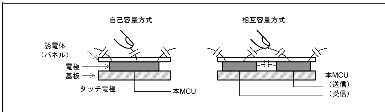
図 44.2 自己容量方式と相互容量方式
