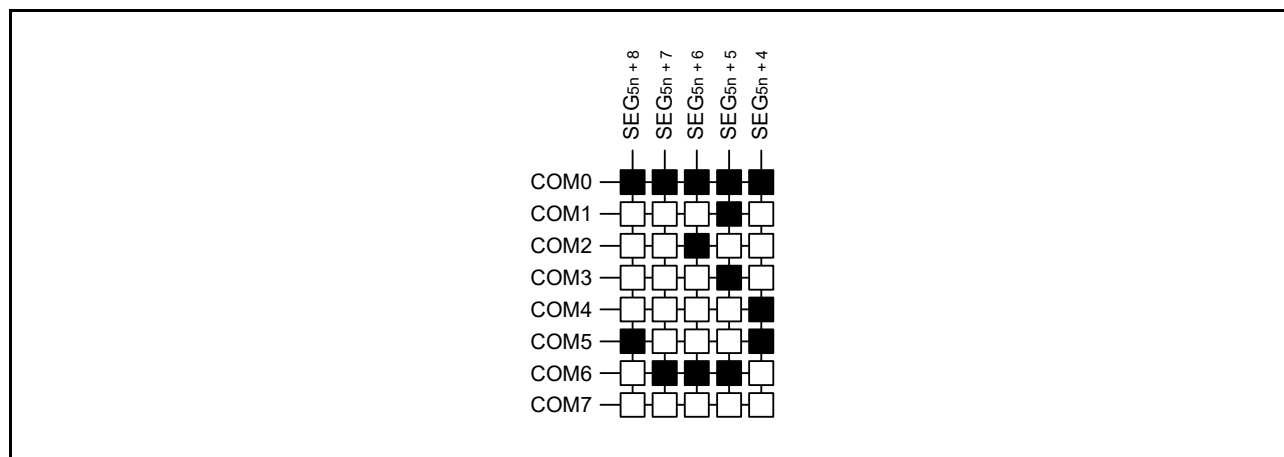
図 48.32 8 時分割 LCD 表示パターンと電極接続
