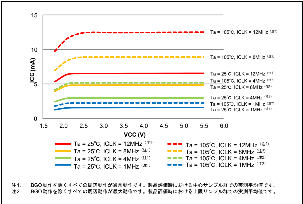
図 50.18 Middle-speed モードにおける電圧依存性 (参考データ)
