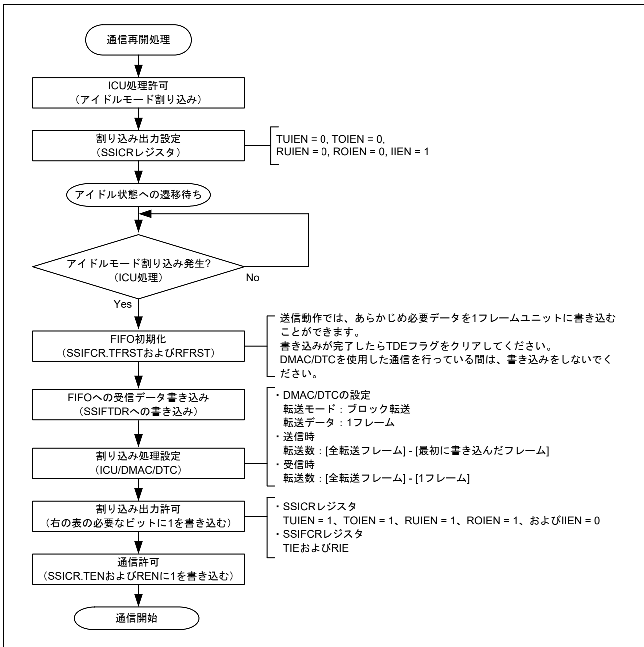
図 35.54 通信再開手順 (CPU 動作)
