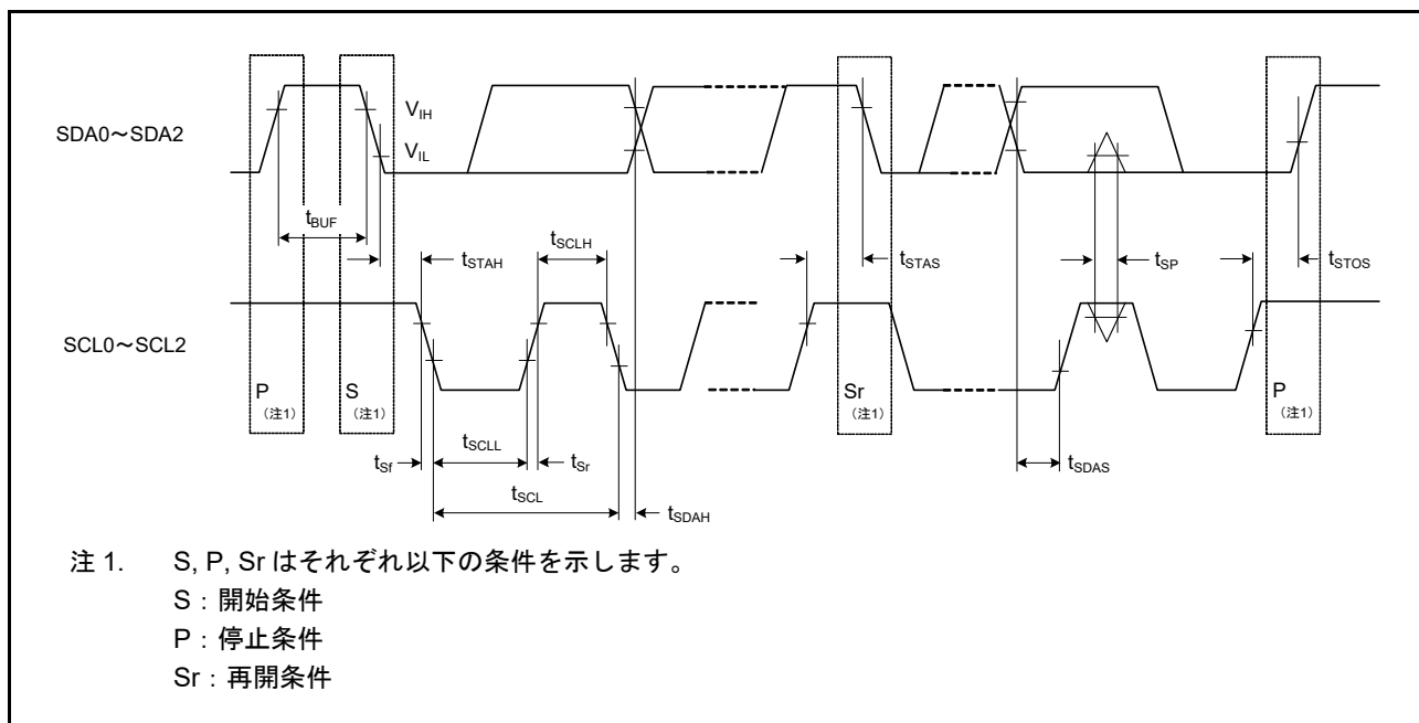
図 50.70 I 2 C バスインタフェース入出カタイミング
