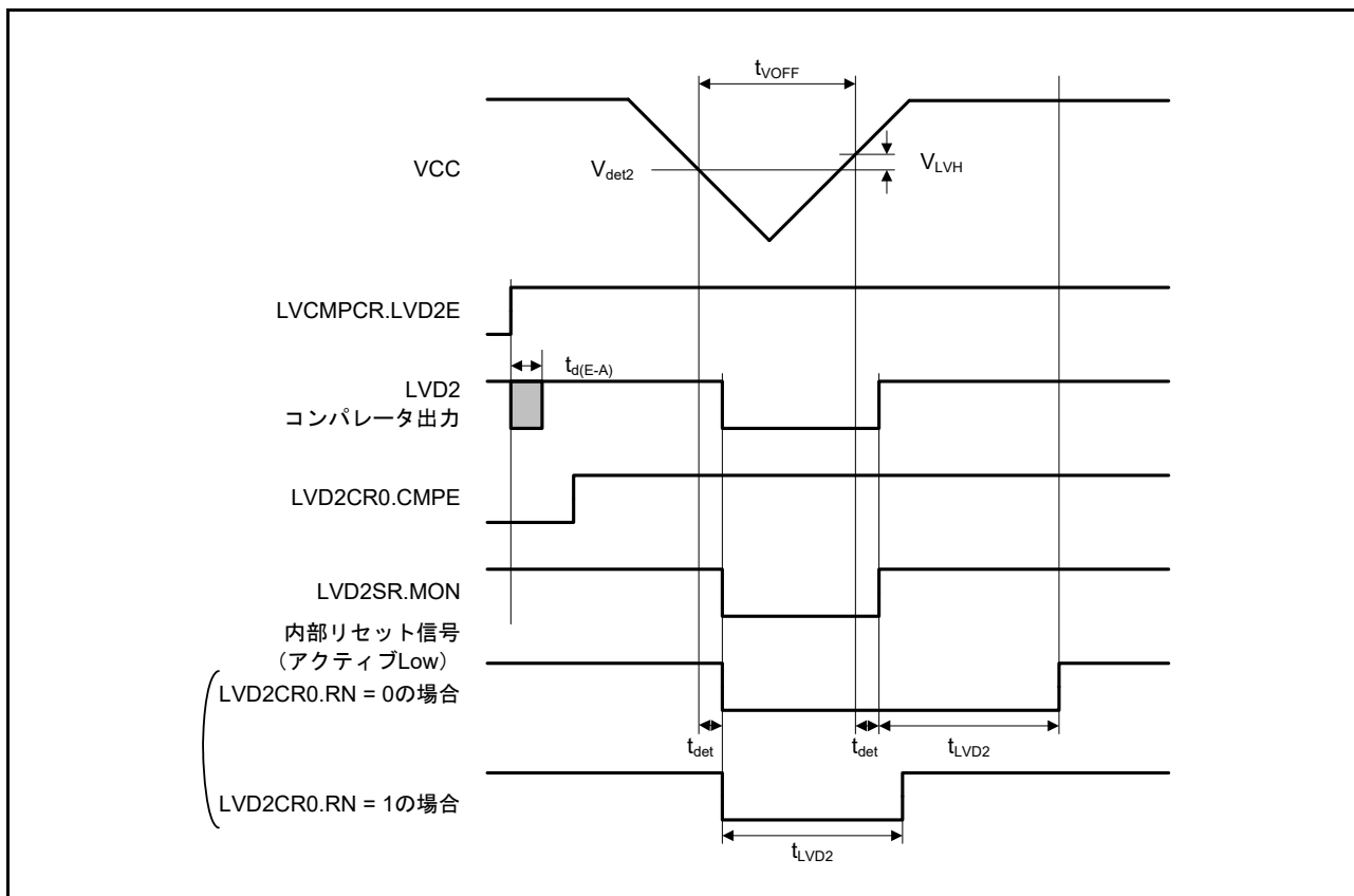
図 50.88 電圧検出回路タイミング ( V_{det2} )
