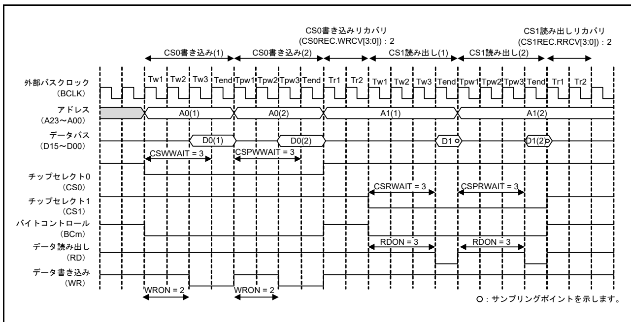
図 15.33 バスアクセスが分割された場合のリカバリサイクルの挿入例 (セパレートバスインタフェースによるページアクセスの場合) (m = 0, 1)
