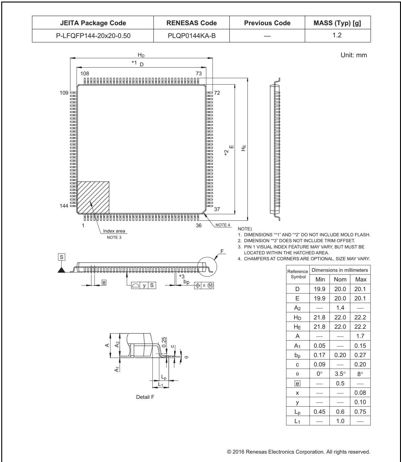
図 2.2 144-pin LQFP
