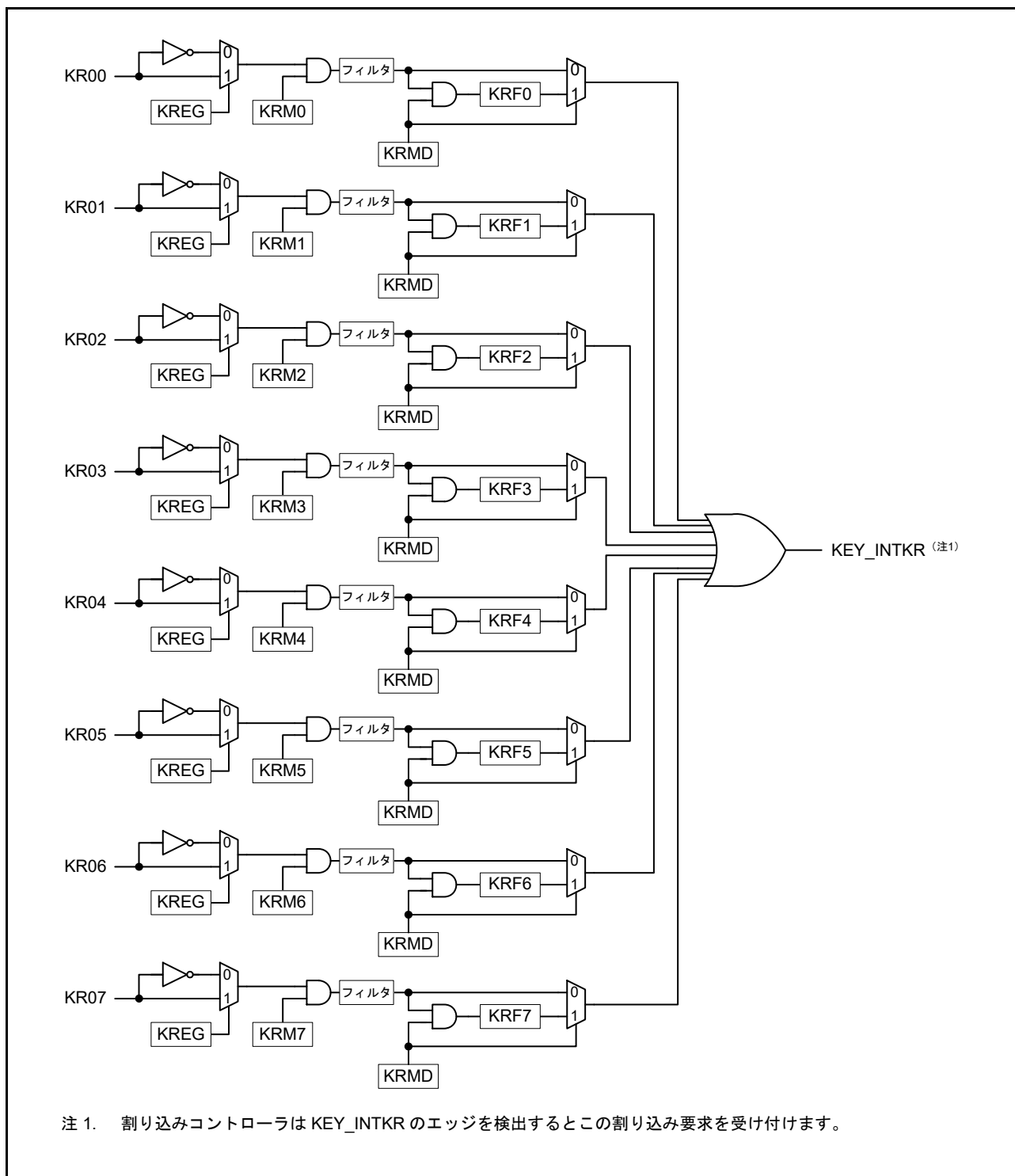
図 21.1 キー割り込み機能のブロック図
