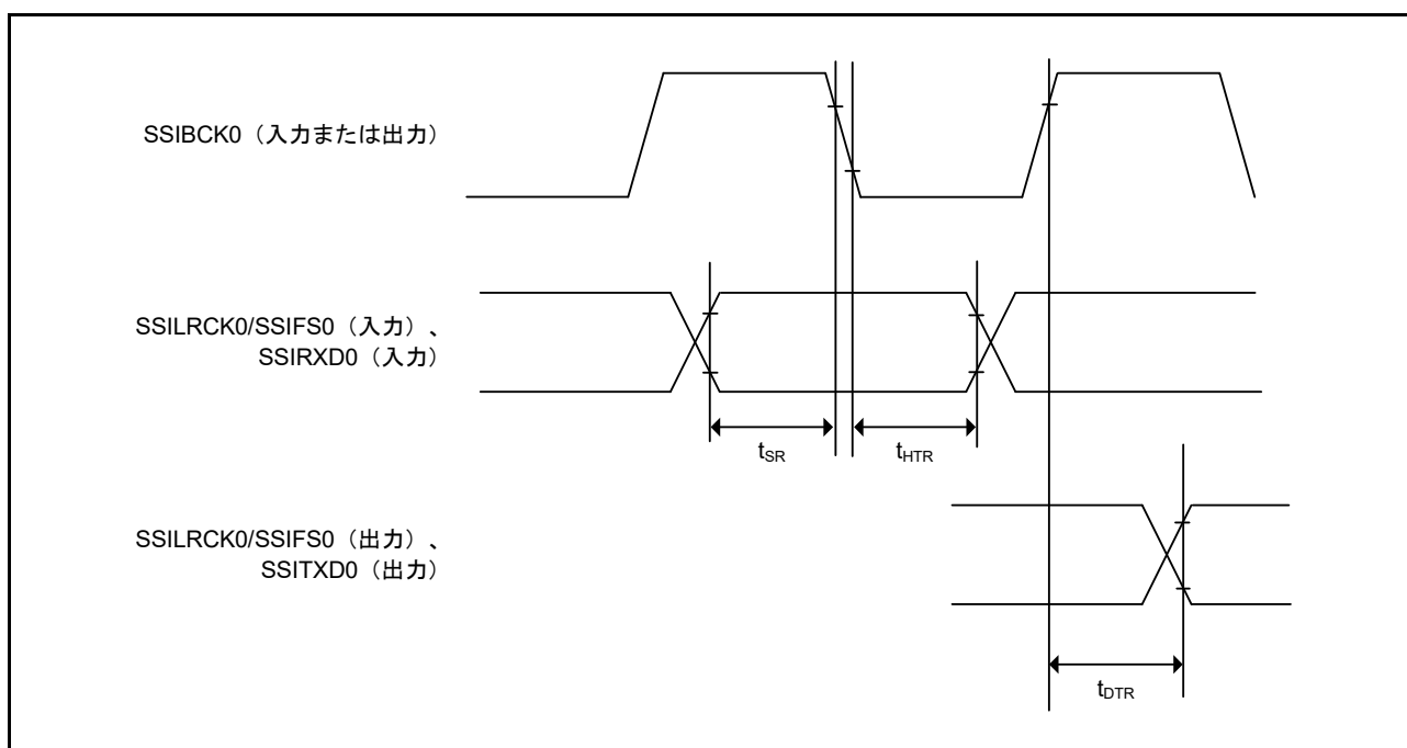
図 50.73 SSIE データ送受信タイミング (SSICR.BCKP = 1)
