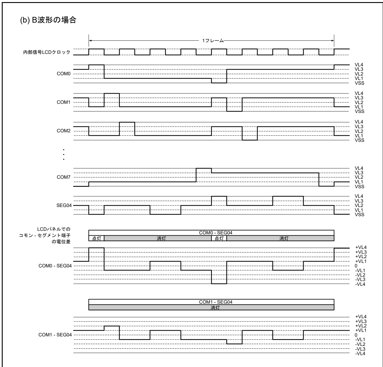
図 48.35 1/4 バイアス法を用いた SEG04 と各コモン信号との間の 4 時分割 LCD 駆動波形例 (2/2)
