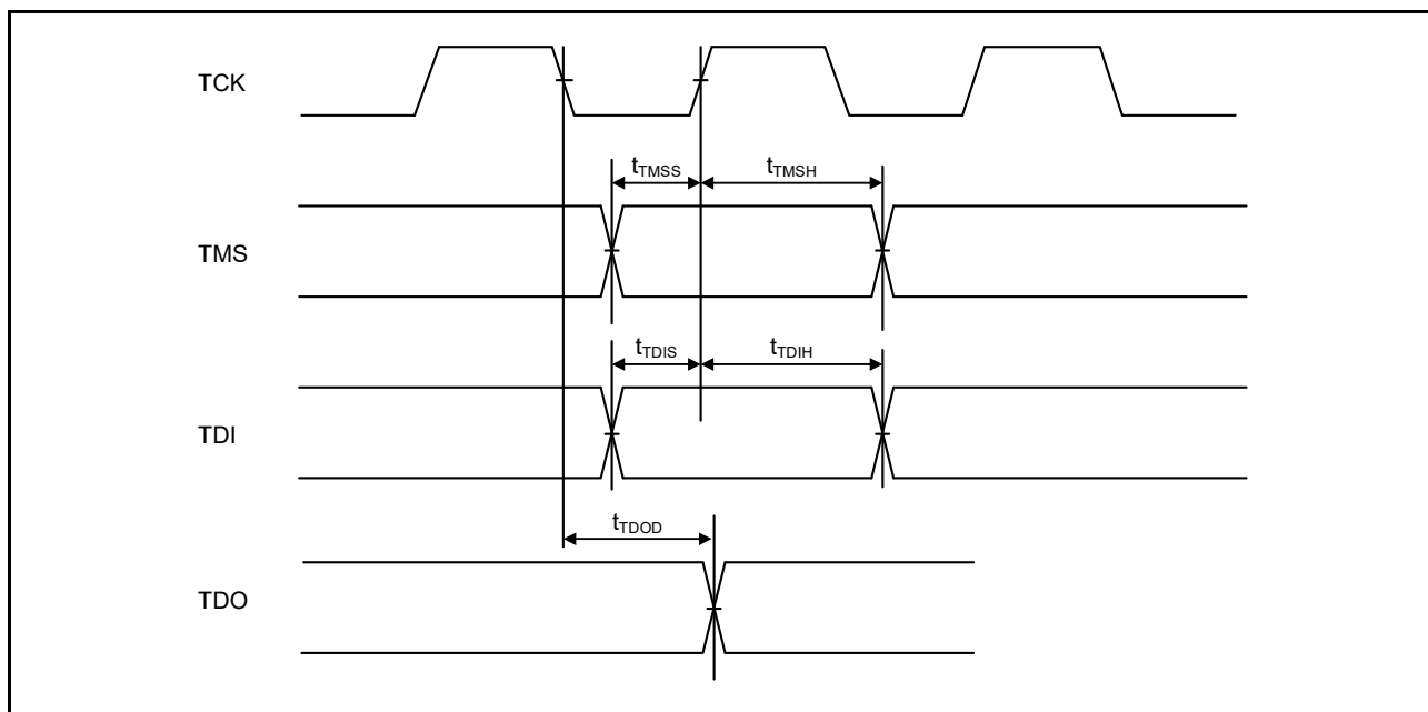
図 50.97 JTAG 入出カタイミング
