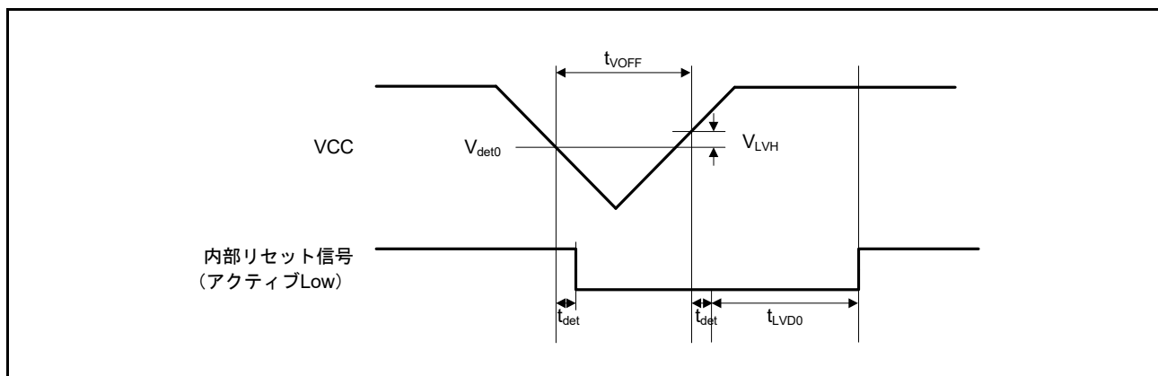
図 50.86 電圧検出回路タイミング ( V_{det0} )
