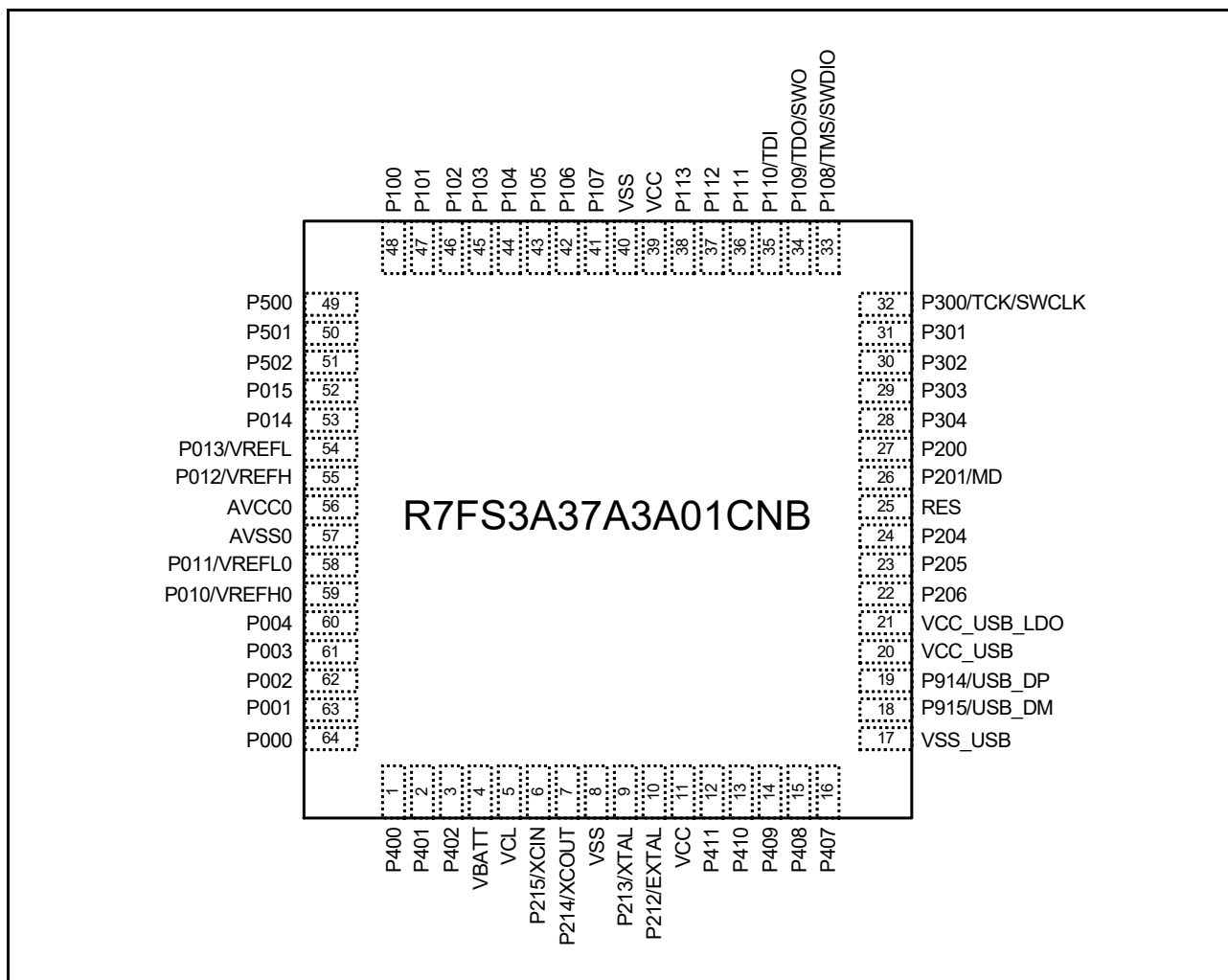
図 1.9 64-pin QFN のピン配置図 (上面透視図)
