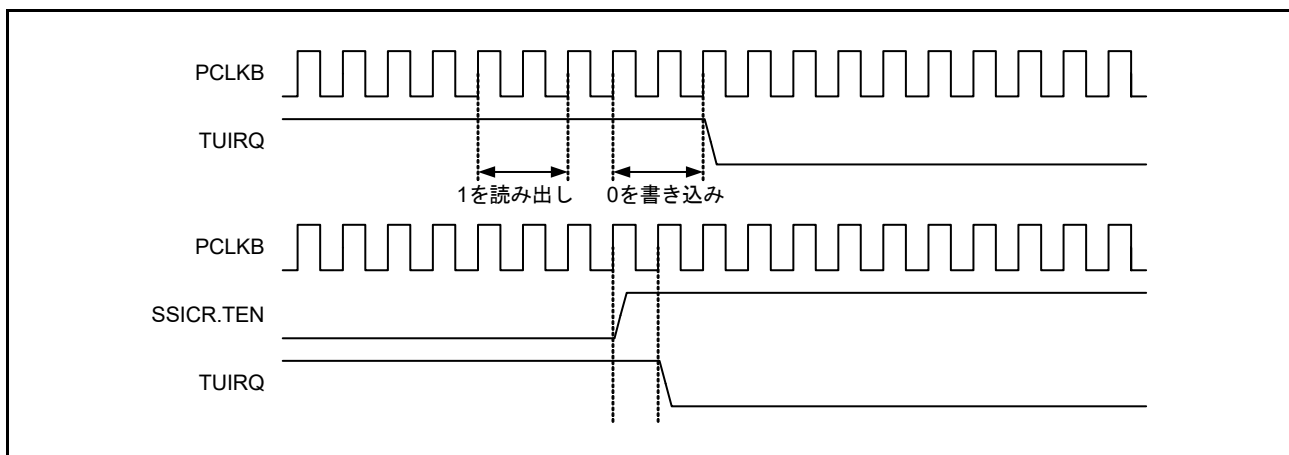
図 35.17 TUIRQ クリアタイミング
