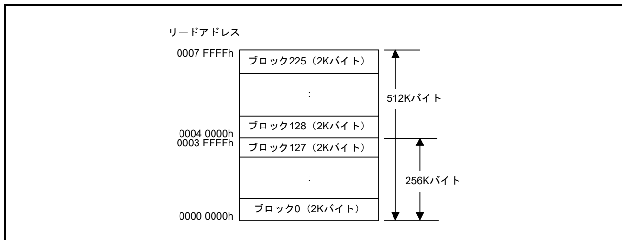
図 47.2 コードフラッシュメモリマッピング
