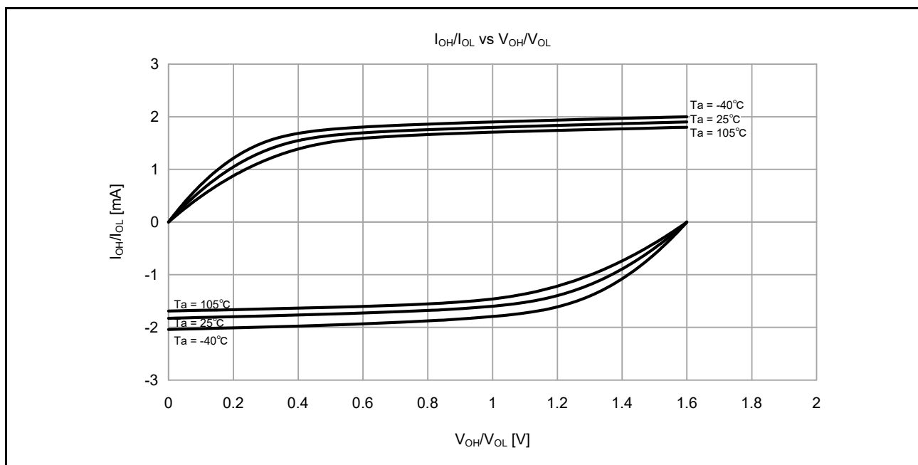
図 50.3 低駆動出力選択時の V_{CC} = 1.6\text{V} での V_{OH}/V_{OL} および I_{OH}/I_{OL} 温度特性 (参考データ)
