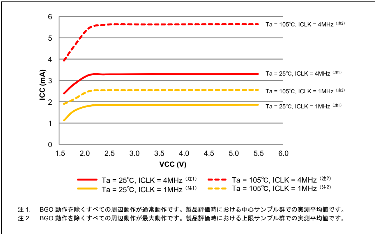
図 50.20 Low-voltage モードにおける電圧依存性 (参考データ)
