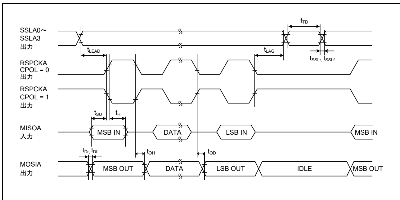
図 50.62 SPI タイミング (マスタ、CPHA = 0) (ビットレート : PCLKA を 2 分周以外に設定)
