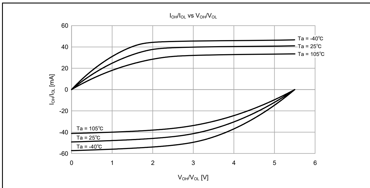
図 50.6 低駆動出力選択時の VCC = 5.5V での V_{OH}/V_{OL} および I_{OH}/I_{OL} 温度特性 (参考データ)
