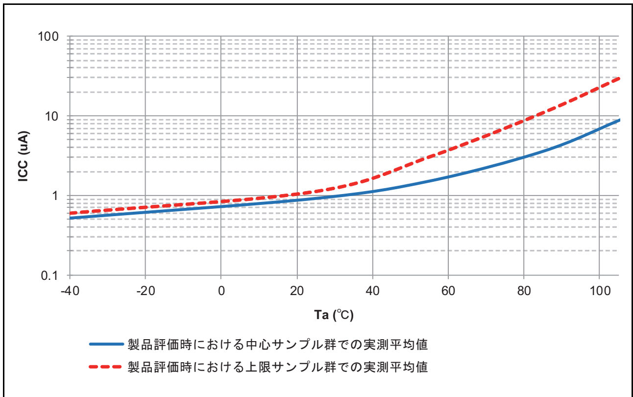
図 50.22 48KB SRAM がオンのソフトウェアスタンバイモード時の温度依存性 (参考データ)
