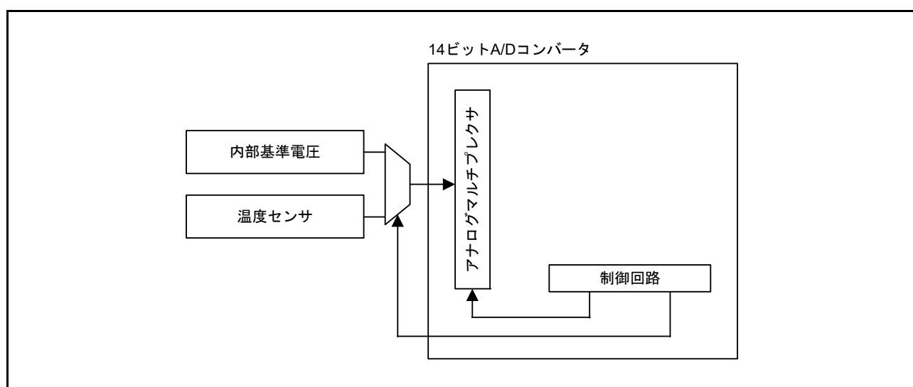
図 40.1 温度センサのブロック図
