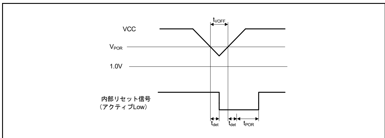
図 50.84 電圧検出リセットタイミング
