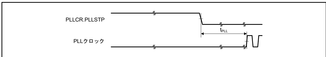
図 50.31 PLL クロック発振開始タイミング (メインクロックの発振安定後に PLL を動作させたとき)
