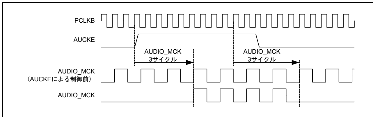
図 35.23 AUDIO_MCK の停止/再開
