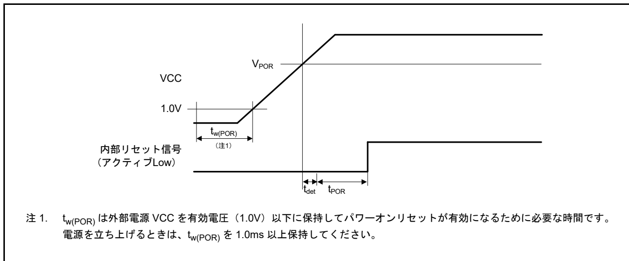
図 50.85 パワーオンリセットタイミング
