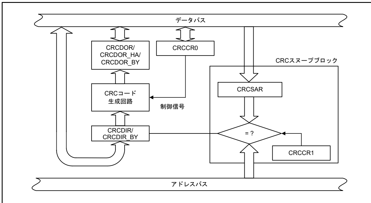
図 34.1 CRC のブロック図
