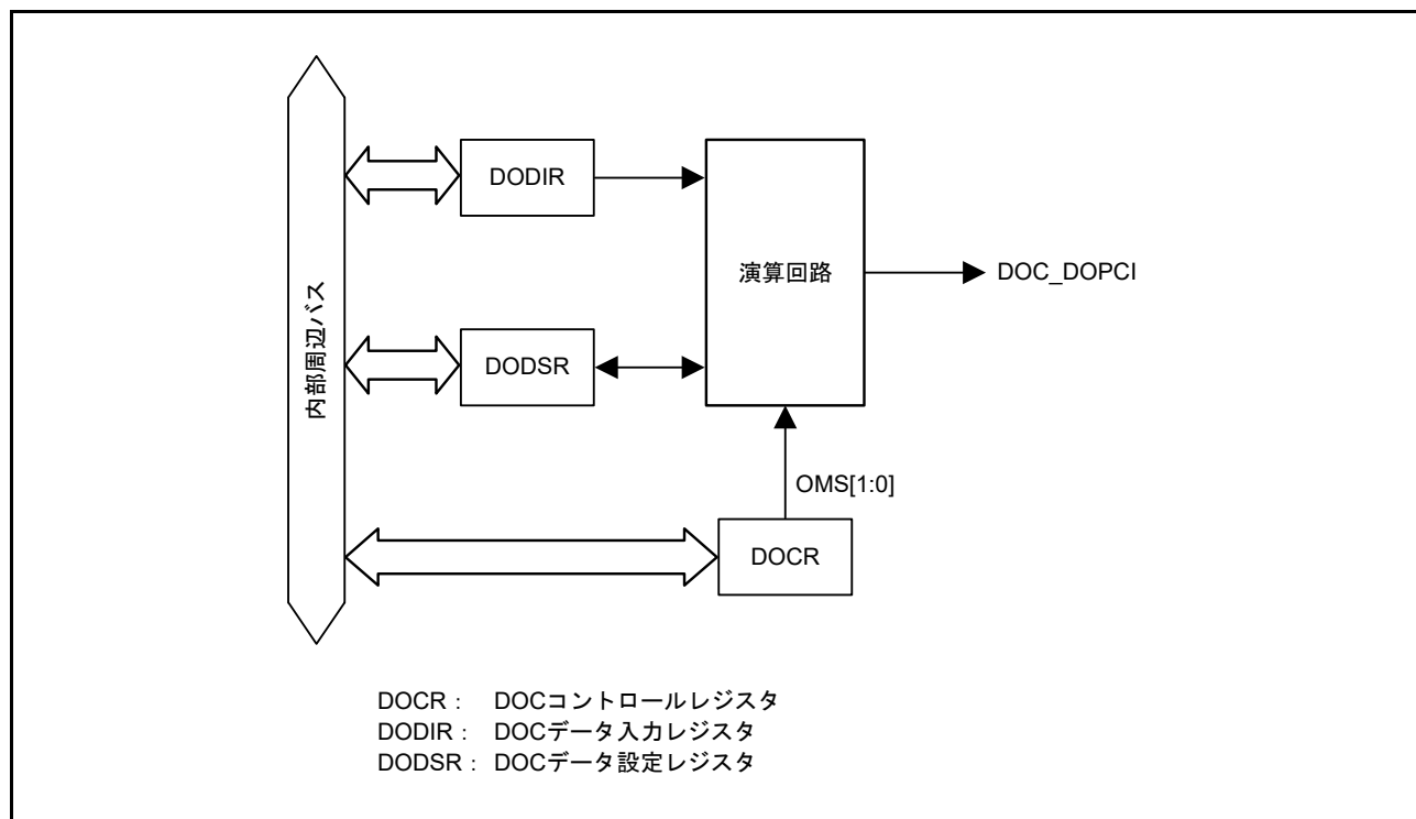
図 45.1 DOC ブロック図
