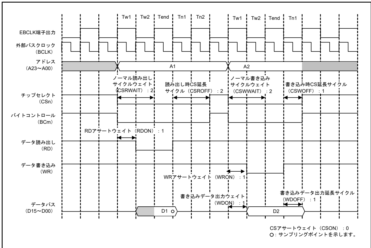
図 15.12 ノーマルアクセスの動作例 (EBCLK 端子出力選択ビットで BCLK の 2 分周を選択した場合) (n = 0 ~ 3, m = 0, 1)
