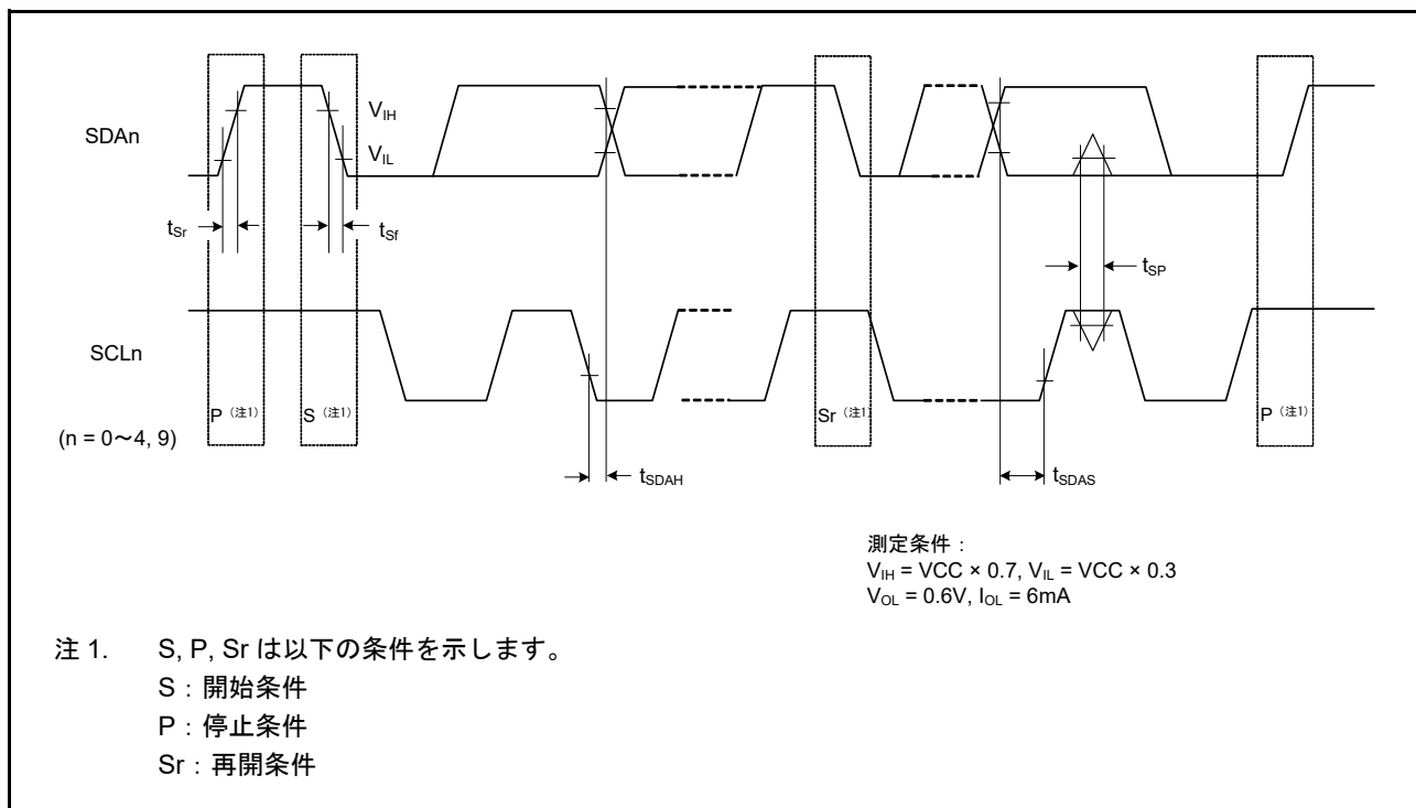
図 50.60 SCI 簡易 IIC モードタイミング
