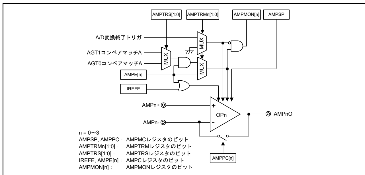
図 41.1 オペアンプのブロック図
