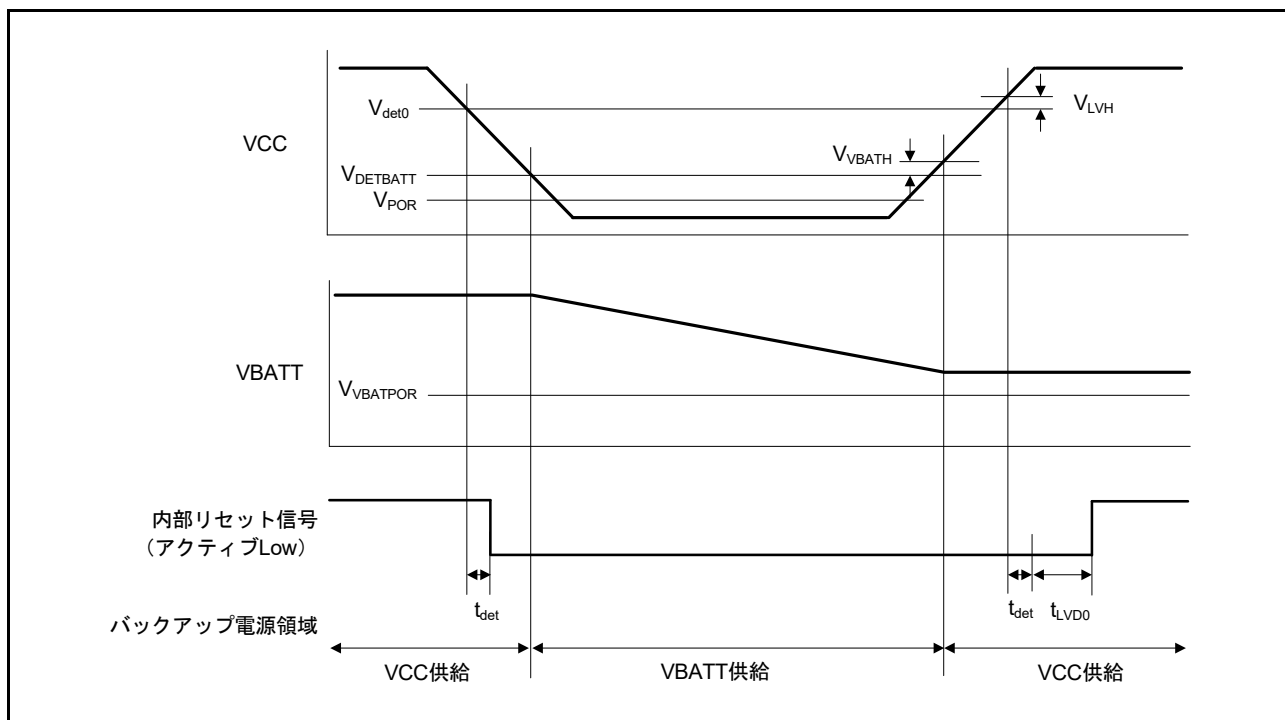
図 50.89 電源切り替えおよびLVD0リセットタイミング
