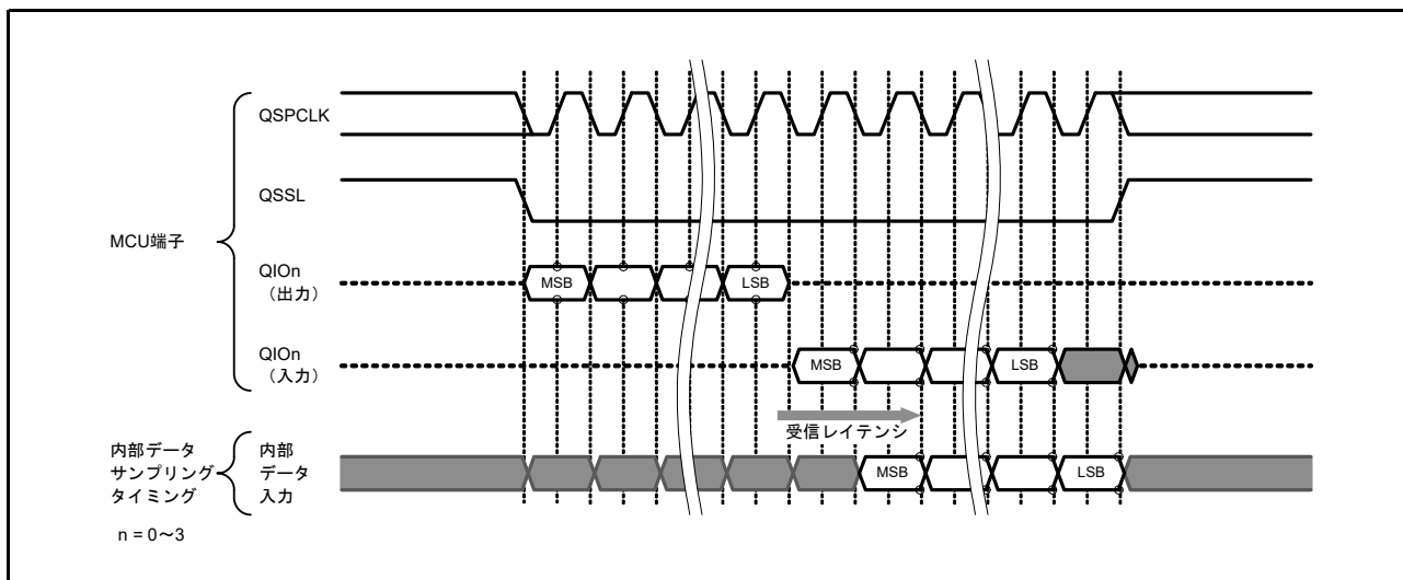
図 33.15 受信レイテンシ
