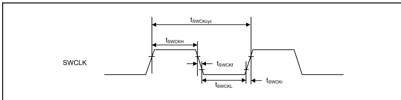
図 50.98 SWD SWCLK タイミング
