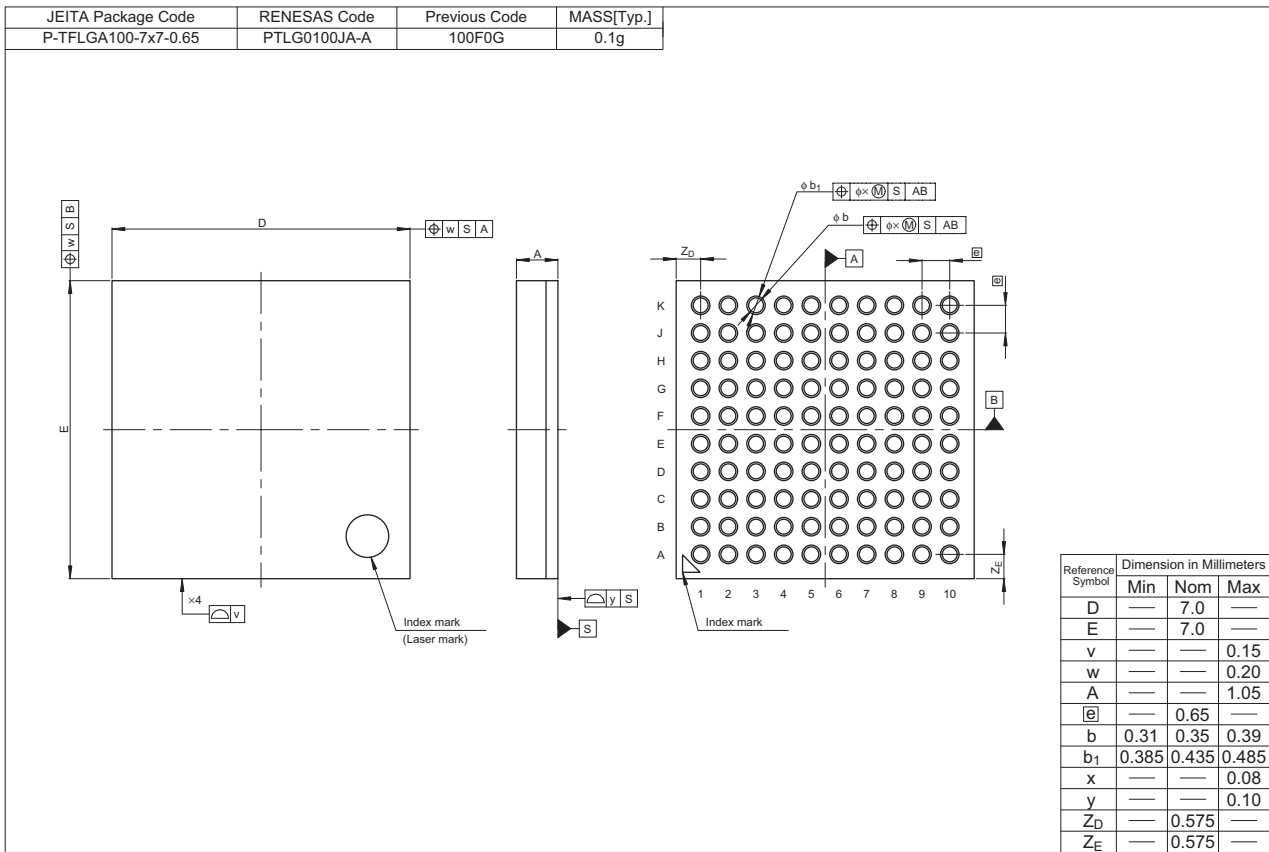
図 2.4 100-pin LGA
