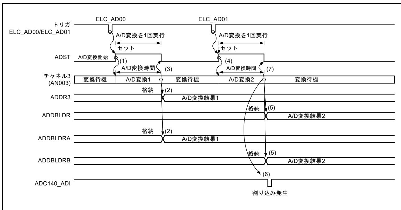
図 38.10 ダブルトリガモードの拡張動作例 (1) (ELC_AD00/ELC_AD01 選択、AN003 を2重化)
