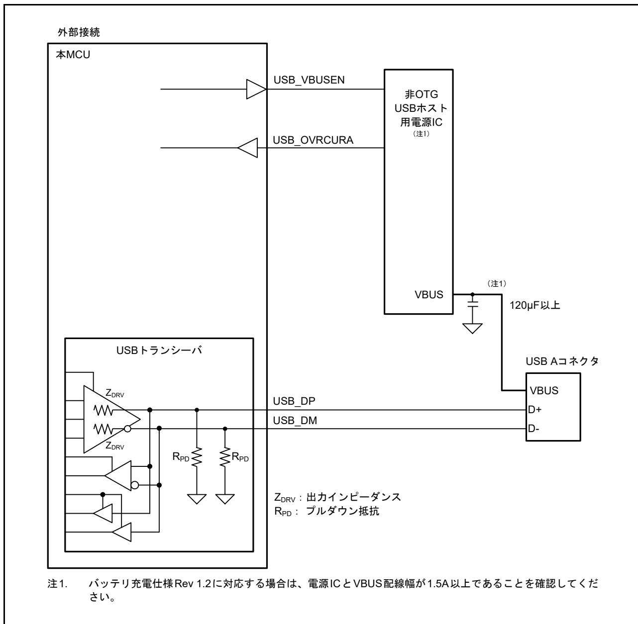
図 28.7 ホスト接続例
