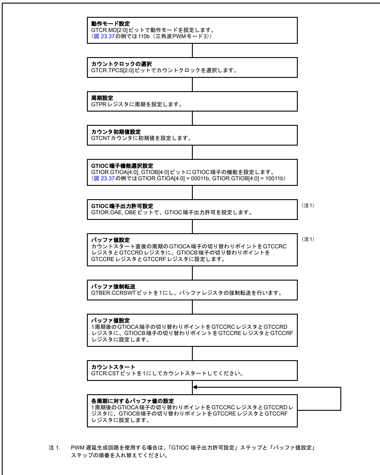
図 23.38 三角波 PWM モード 3 の設定例
