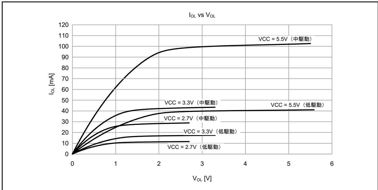
図 50.16 Ta = 25 °Cでの V OH /V OL および I OH /I OL 電圧特性
