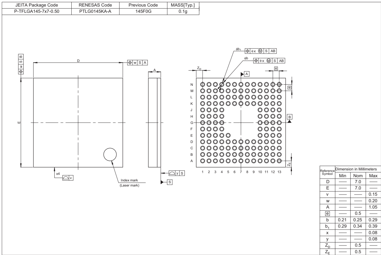
図 2.1 145-pin LGA
