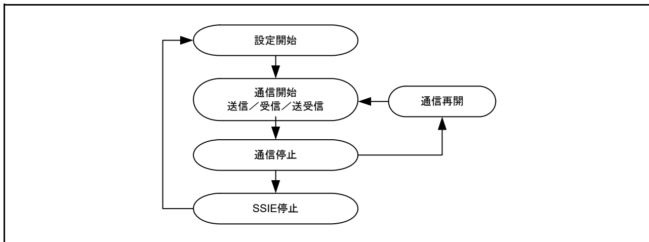
図 35.48 SSIE 通信動作
