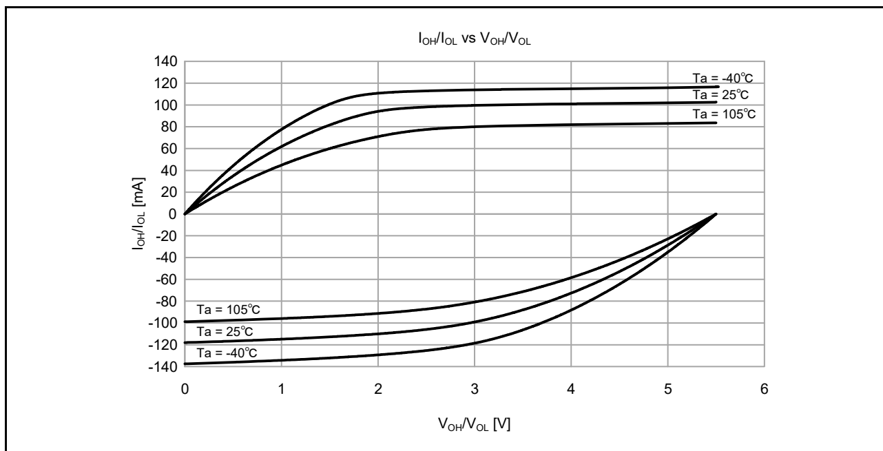
図 50.11 中駆動出力選択時の V_{CC} = 5.5\text{V} での V_{OH}/V_{OL} および I_{OH}/I_{OL} 温度特性 (参考データ)
