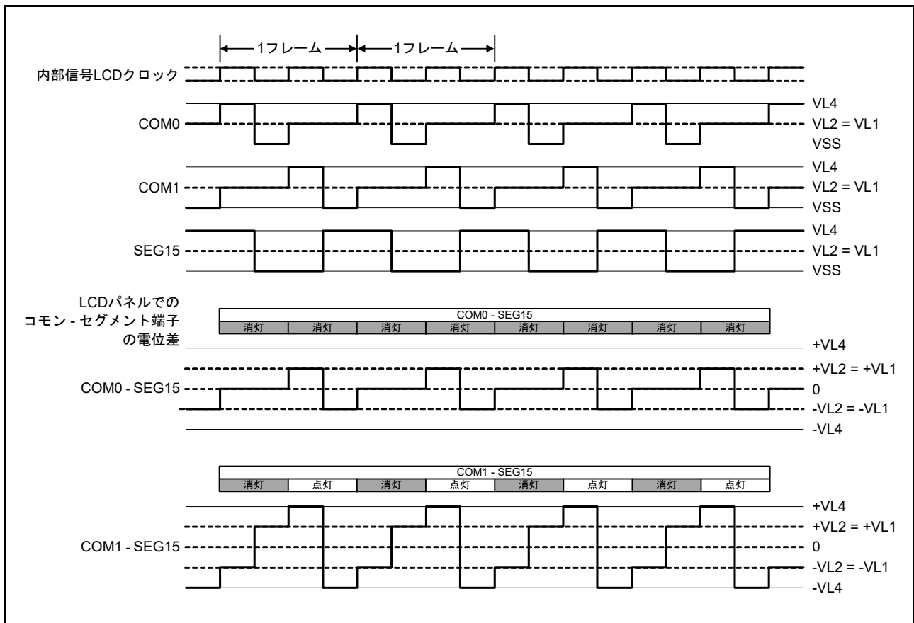
図 48.23 SEG15 と各コモン信号との間の 2 時分割 LCD 駆動波形例 (1/2 バイアス法)
