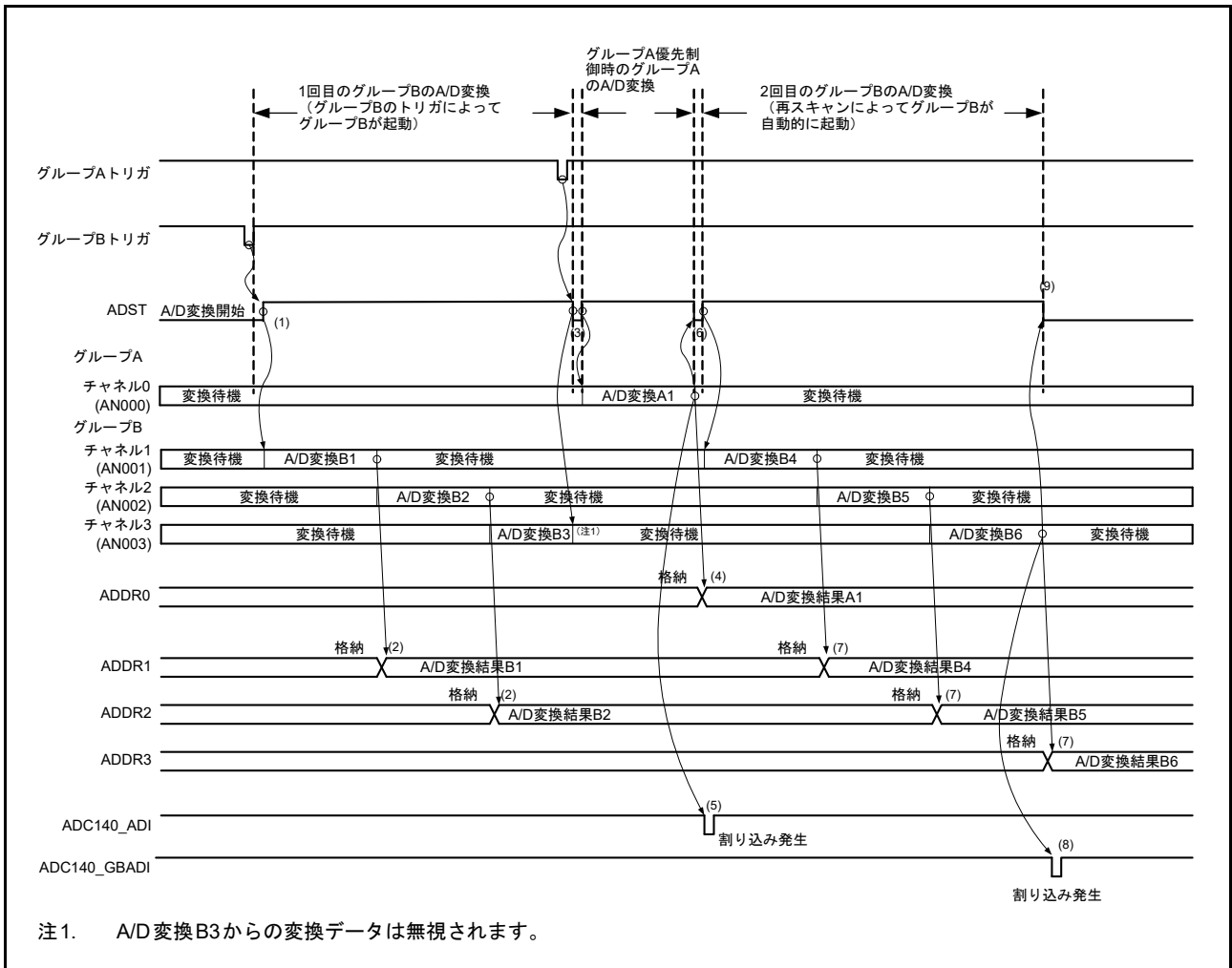
図 38.16 グループ A 優先制御の動作例 (1) (ADGSPCR.GBRSCN = 1, ADGSPCR.GBRP = 0 の場合)
