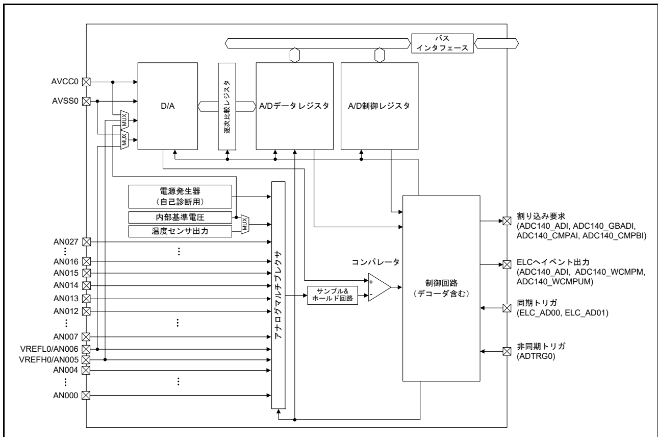
図 38.1 ADC14 のブロック図
