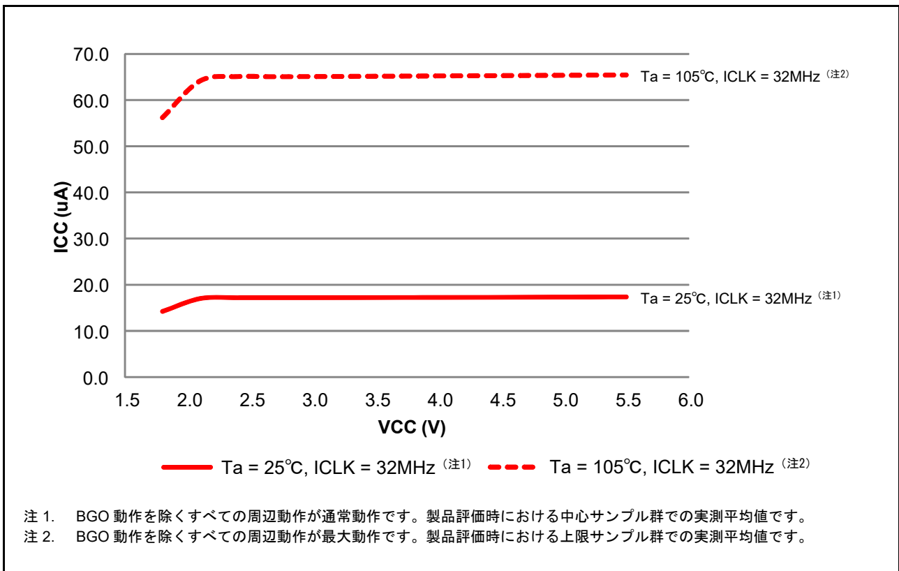
図 50.21 Subosc-speed モードにおける電圧依存性 (参考データ)
