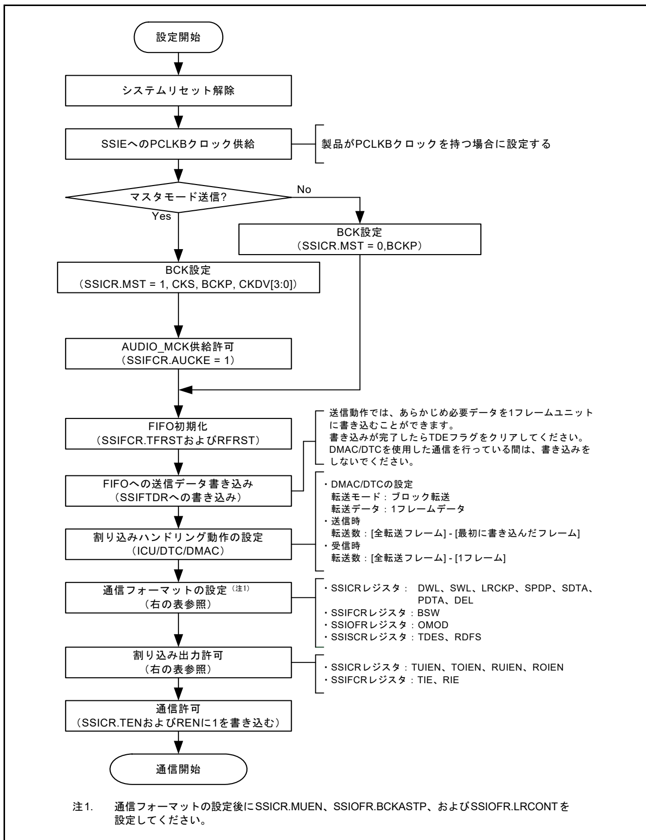
図 35.49 通信開始手順 (CPU 動作手順)
