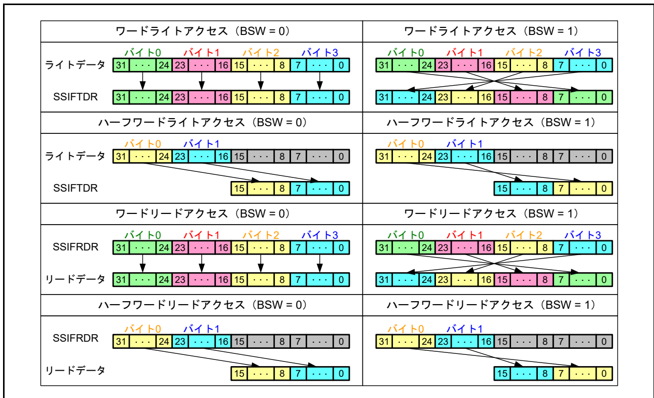
図 35.22 バイトスワップの動作例
