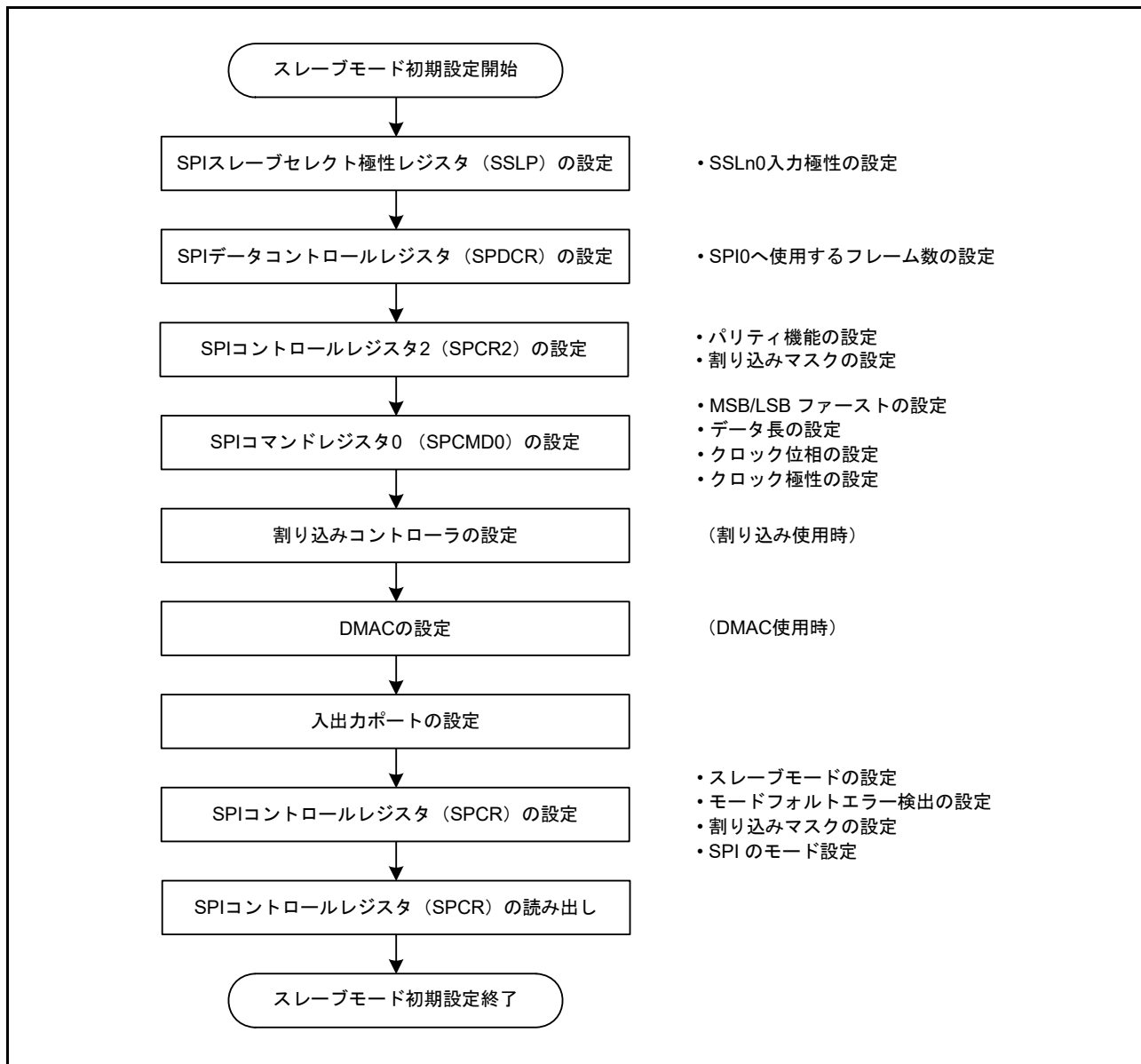
図 32.47 スレーブモード時の SPI 動作の初期化フロー例
