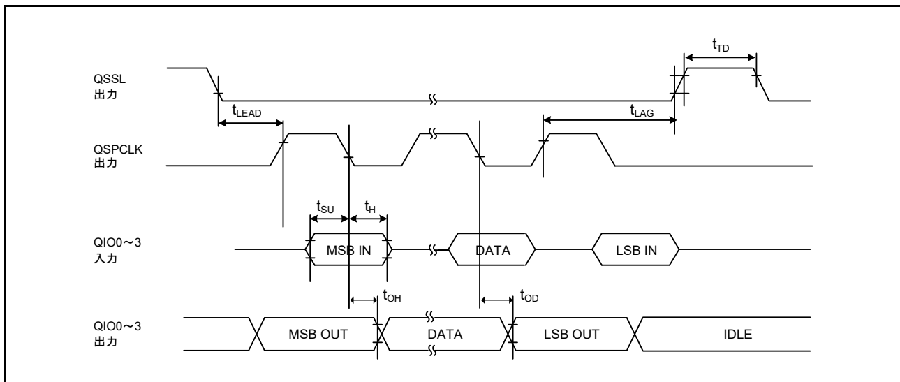
図 50.69 送受信タイミング
