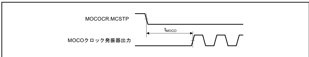
図 50.33 MOCO クロック発振開始タイミング
