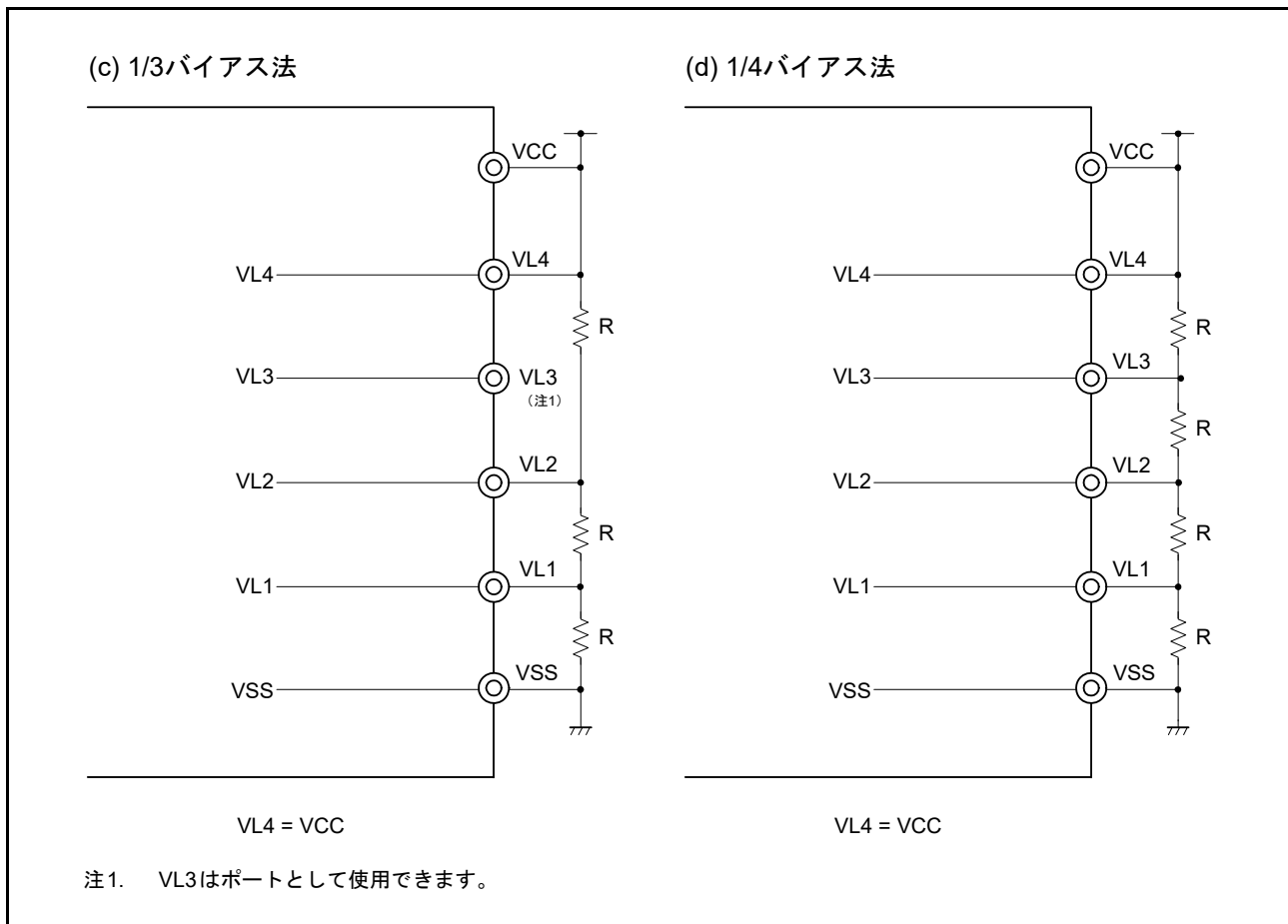
図 48.10 LCD 駆動電源の接続例（外部抵抗分割方式）(2/2)
