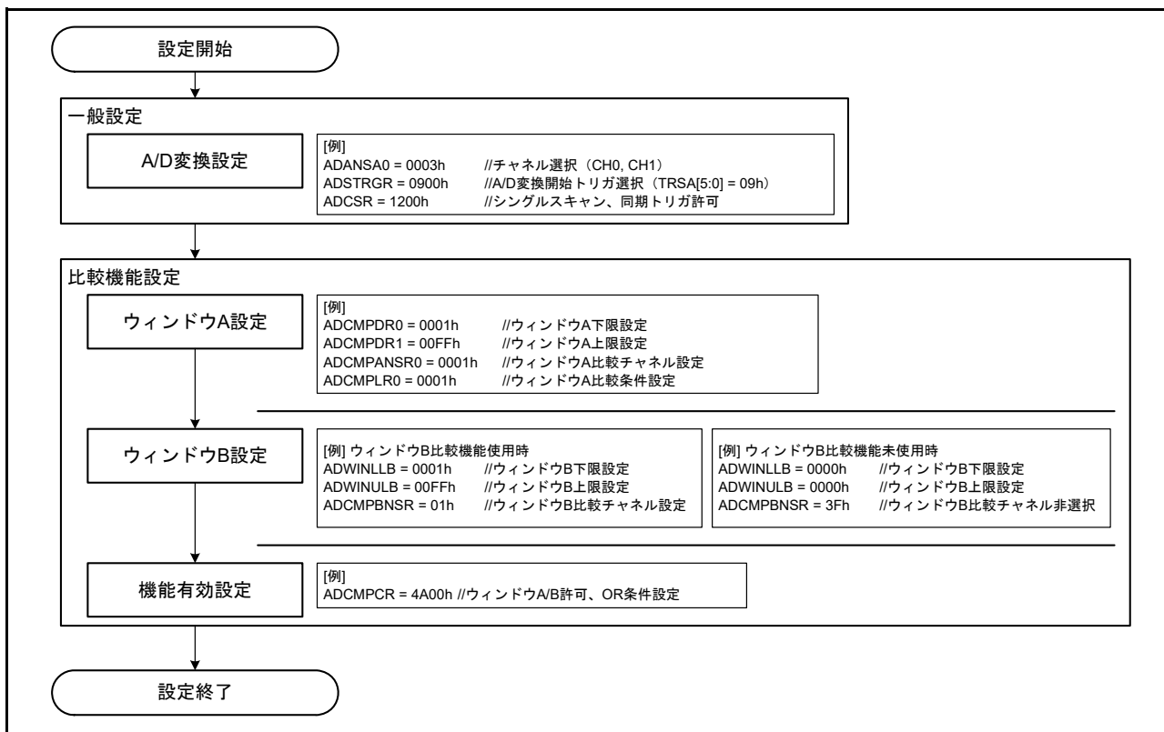
図 38.22 コンペア機能のイベント出力使用時の設定例
