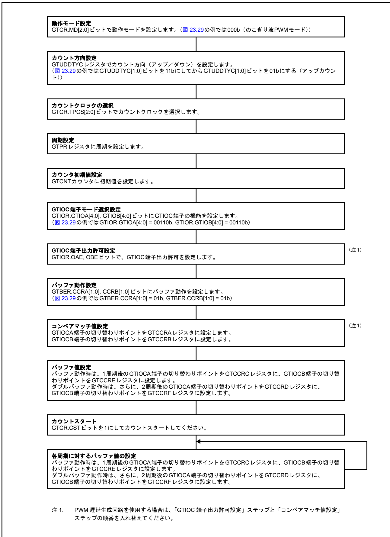
図 23.30 のこぎり波 PWM モードの設定例
