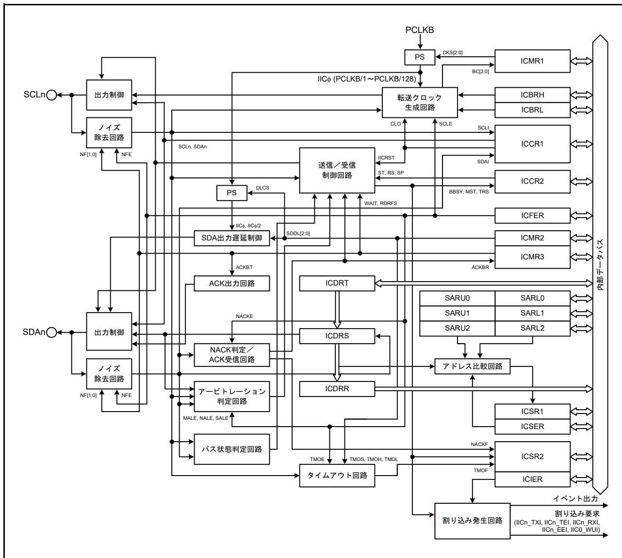
図 30.1 IIC のブロック図
