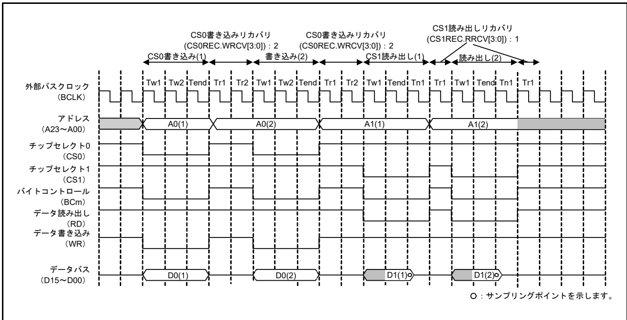
図 15.32 バスアクセスが分割された場合のリカバリサイクルの挿入例 (セパレートバスインタフェースによるノーマルアクセスの場合) (m = 0, 1)
