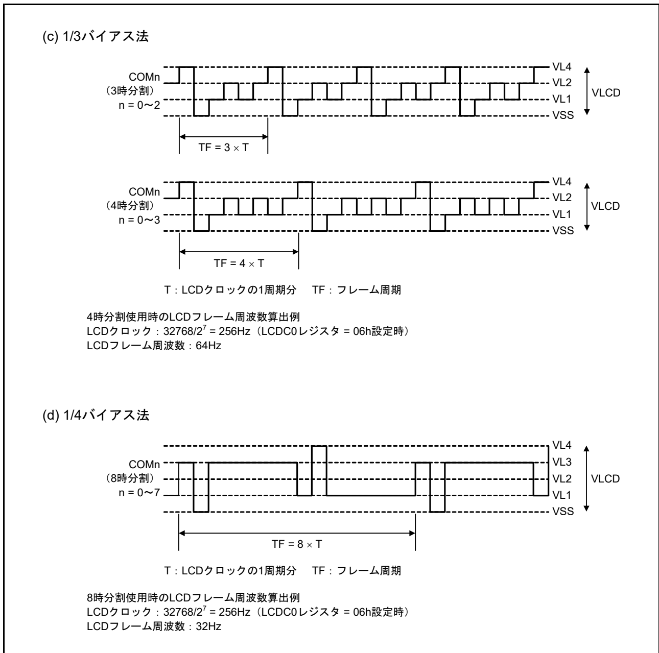
図 48.14 コモン信号波形 (2/2)
