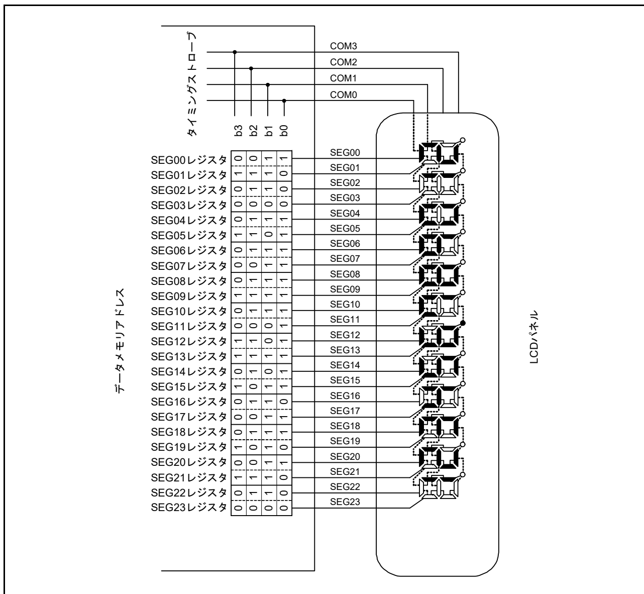
図 48.29 4 時分割 LCD パネルの接続例
