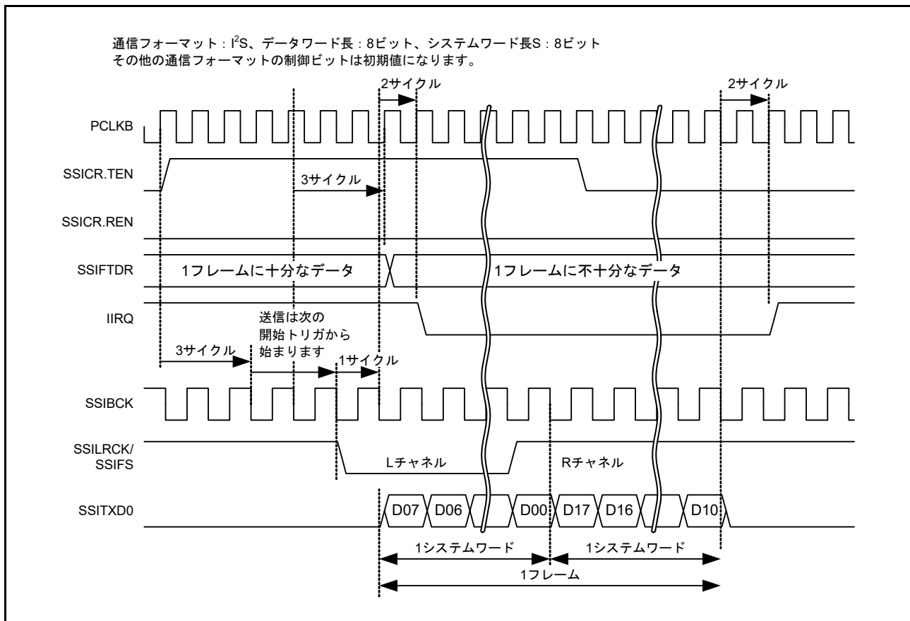
図 35.12 IIRQ 設定タイミング (送信)
