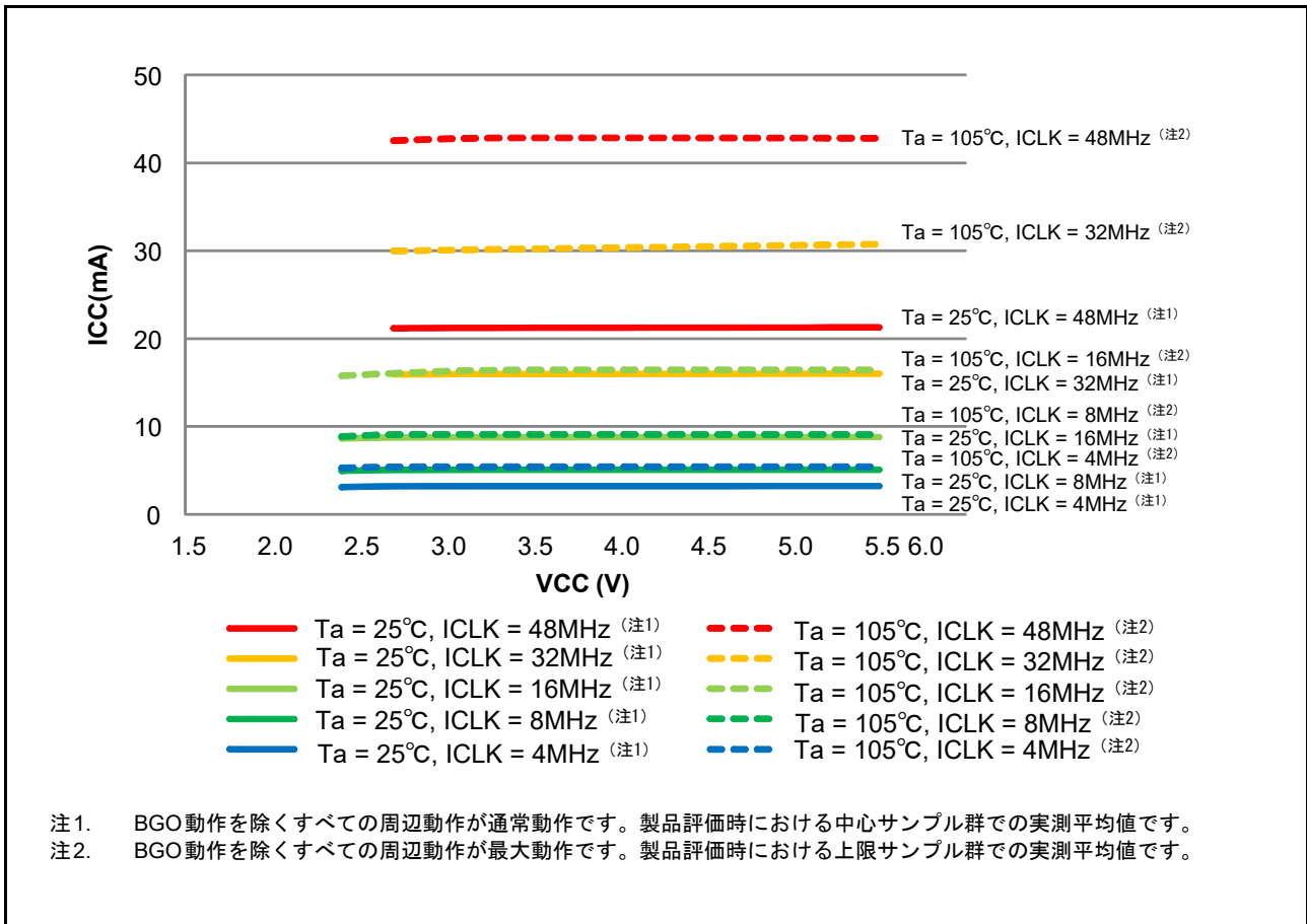
図 50.17 High-speed モードにおける電圧依存性 (参考データ)
