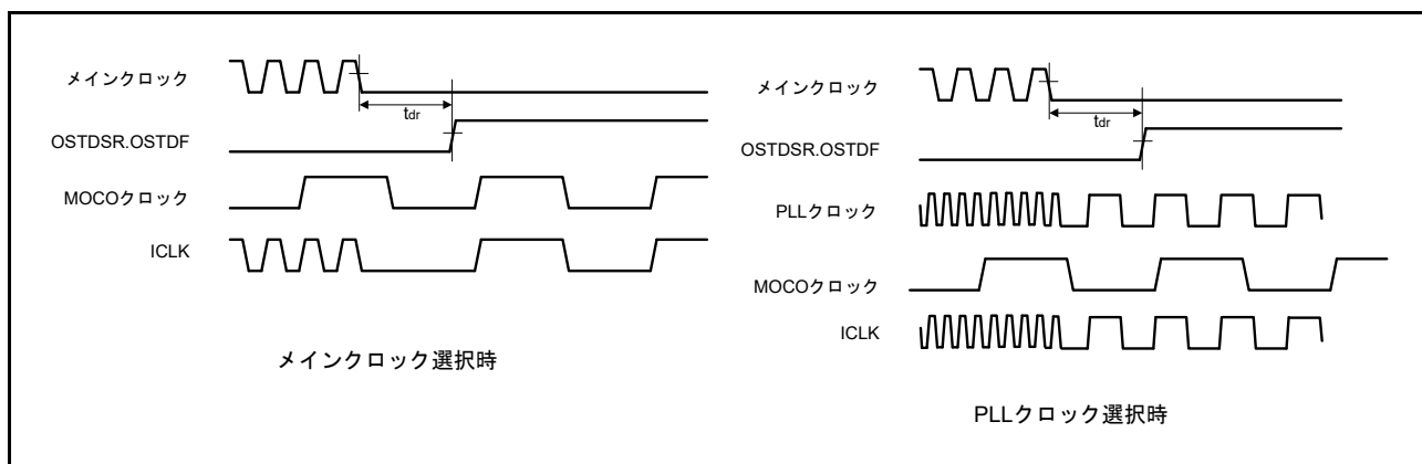
図 50.83 発振停止検出タイミング
