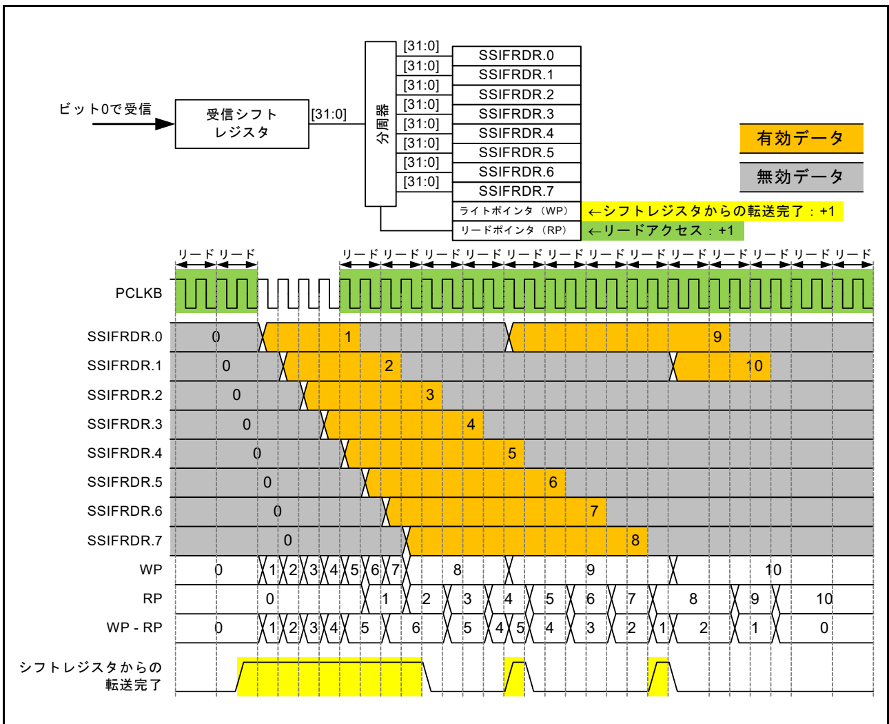
図 35.30 受信 FIFO データレジスタと受信シフトレジスタの構成例および FIFO 動作例
