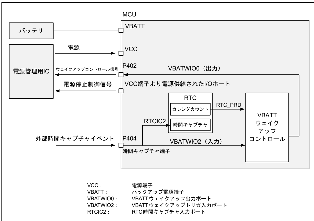
図 12.5 VBAT ウェイクアップコントロール機能の応用例
