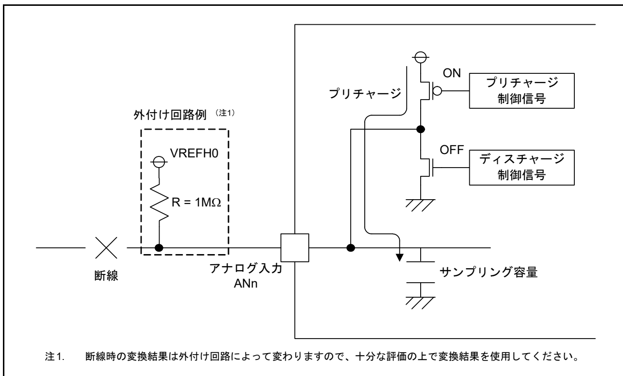
図 38.27 プリチャージを選択した場合の断線検出例
