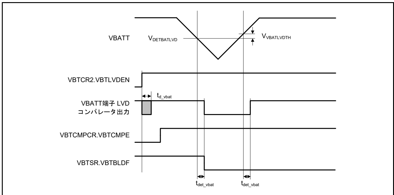
図 50.91 VBATT 端子電圧検出回路タイミング
