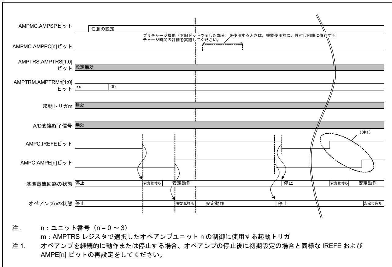
図 41.3 オペアンプの制御動作 (ソフトウェアトリガモードによる制御) (ソフトウェアトリガモードによって基準電流回路およびオペアンプを起動/停止する場合)
