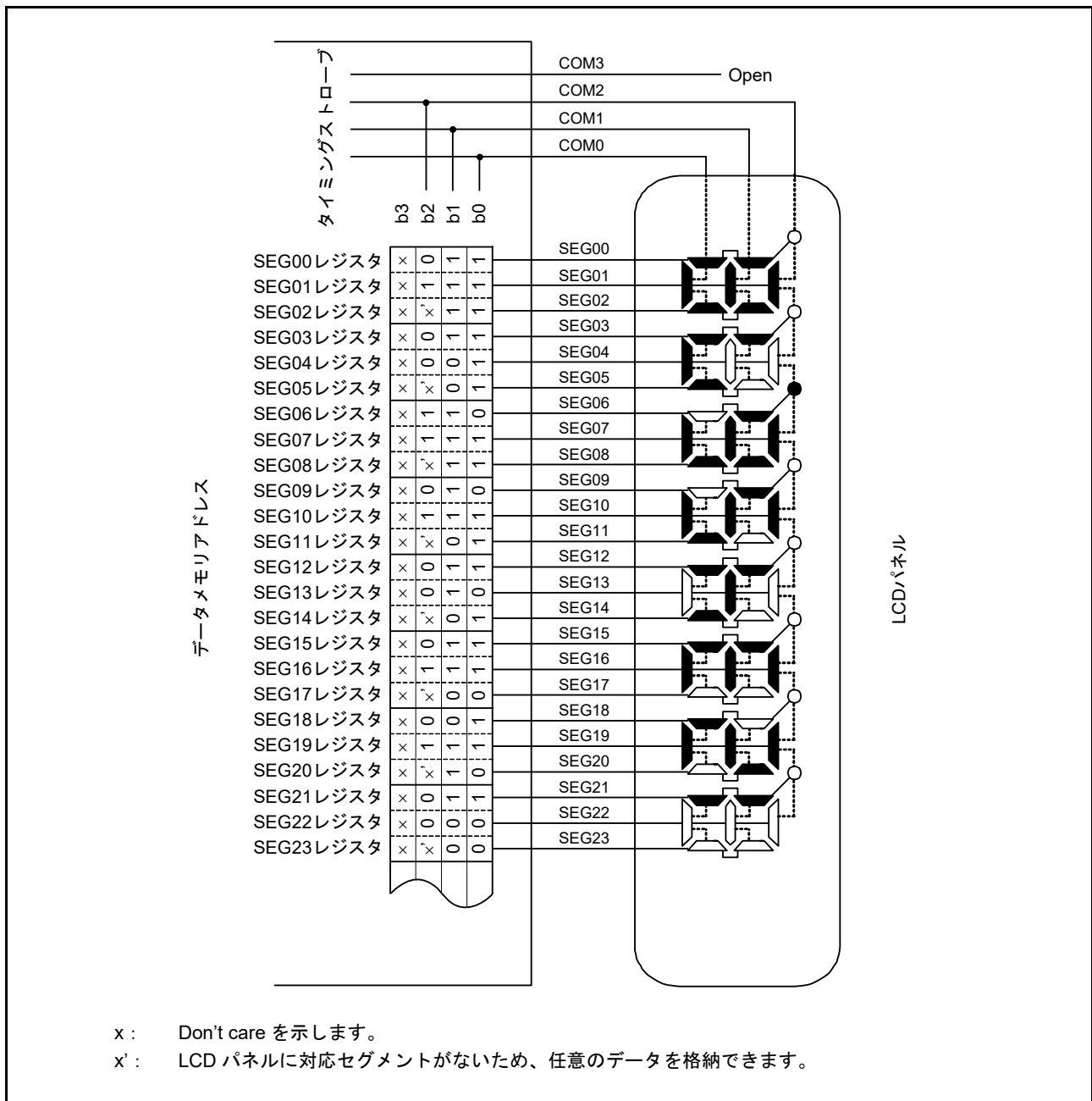
図 48.25 3 時分割 LCD パネルの接続例
