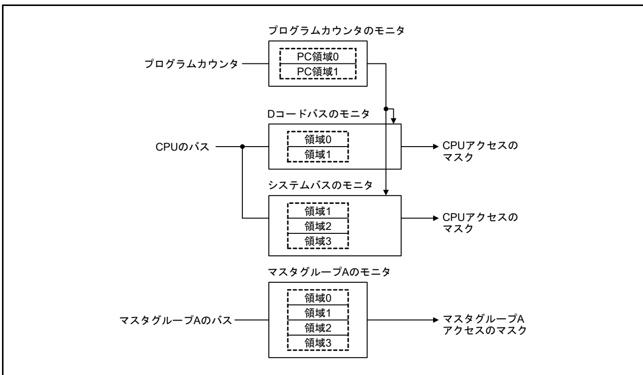
図 16.10 セキュリティ MPU のブロック図
