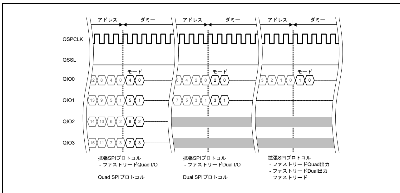
図 33.33 XIP モード制御データ
