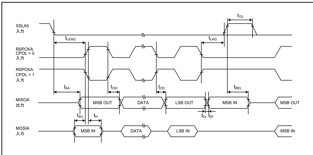
図 50.66 SPI タイミング (スレーブ、CPHA = 0)
