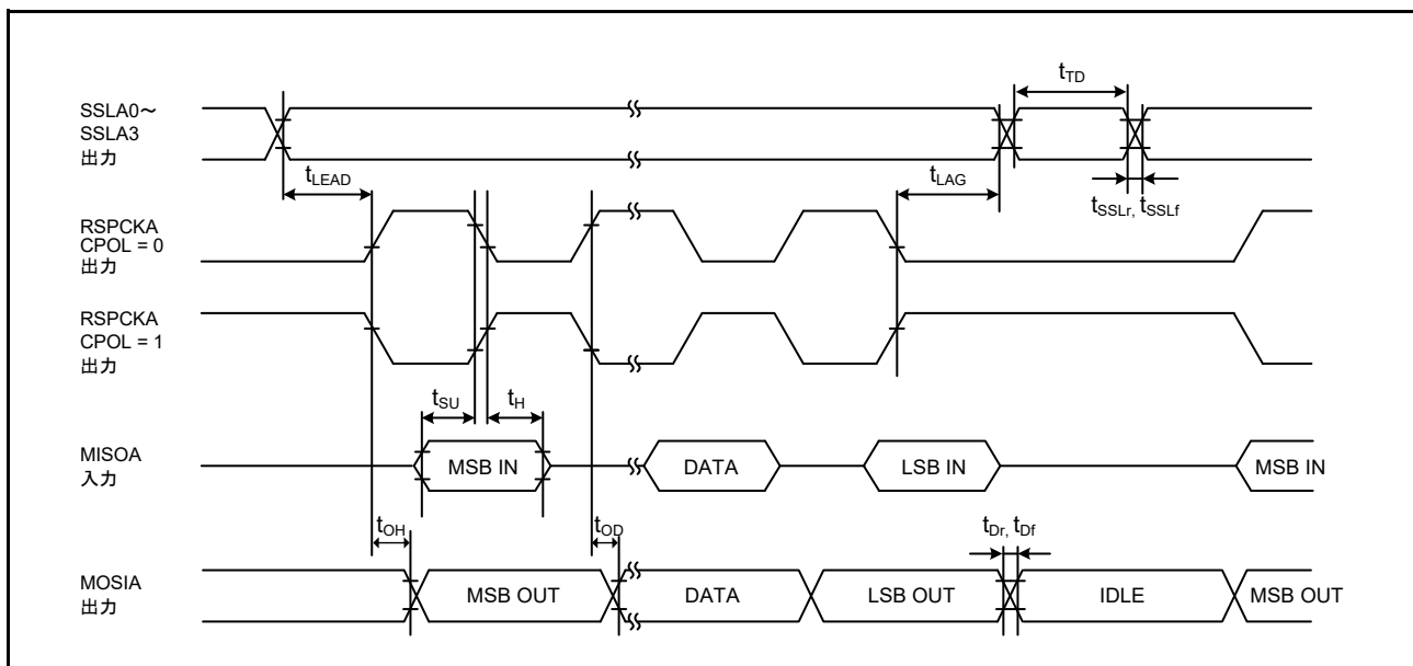
図 50.64 SPI タイミング (マスタ、CPHA = 1) (ビットレート : PCLKA を 2 分周以外に設定)
