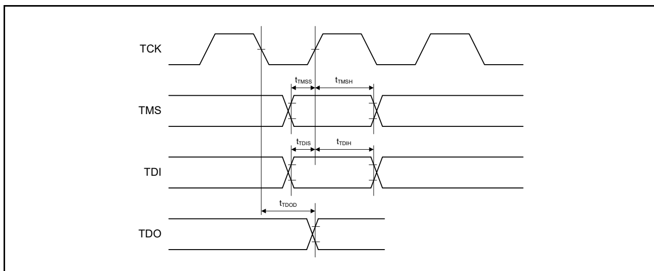
図 50.94 バウンダリスキャン入出力タイミング
