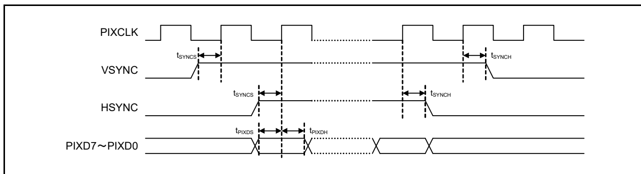
図 55.76 PDC AC タイミング
