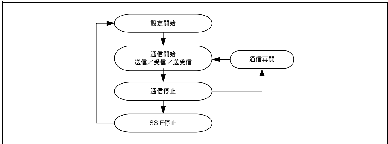
図 39.52 SSIE 通信動作
