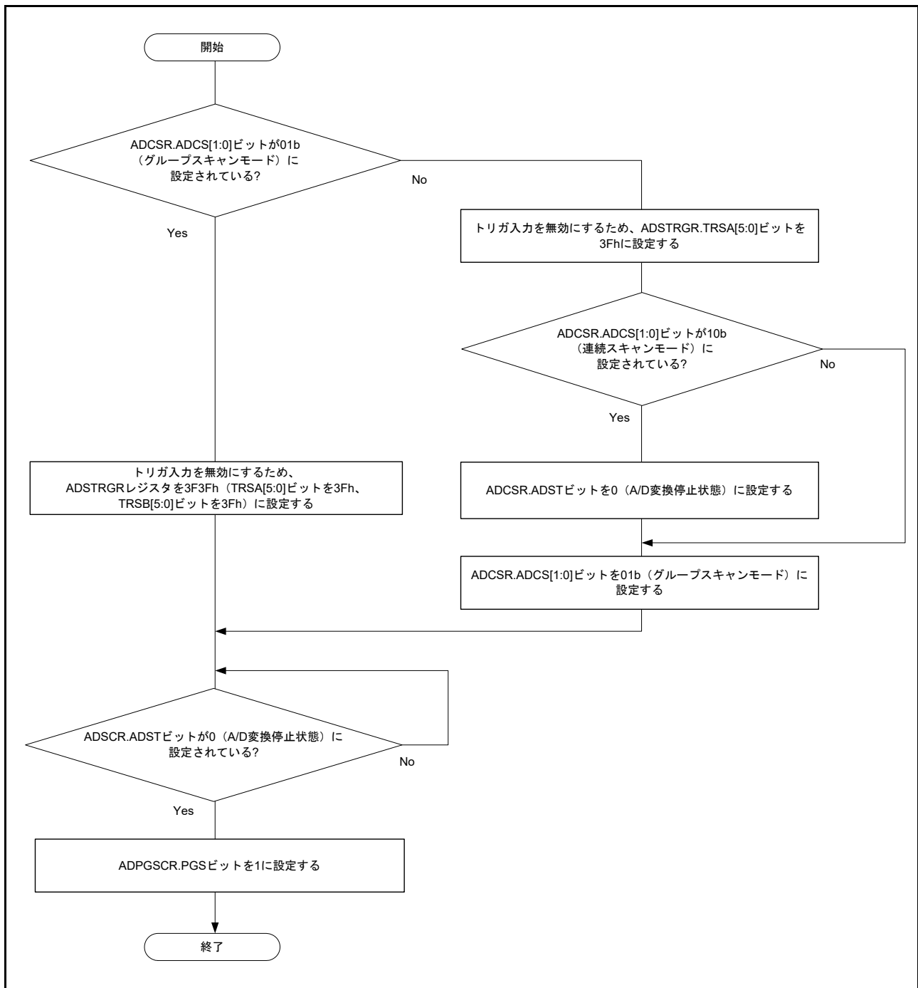
図 45.25 ADPGSCR.PGS ビット設定時のフロー
