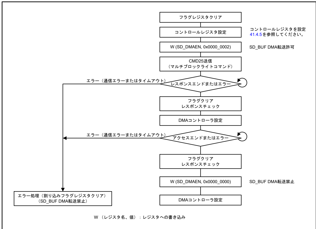
図 41.24 SD_BUF_DMA ライト動作の例
