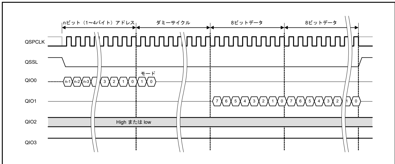
図 37.18 XIP モード時のファストリードバスサイクル
