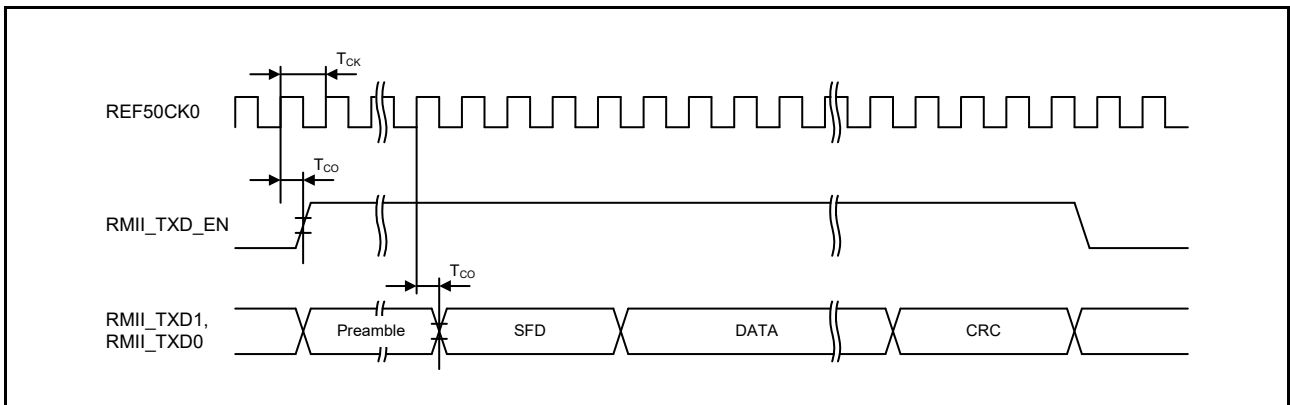
図 55.65 RMII 送信タイミング
