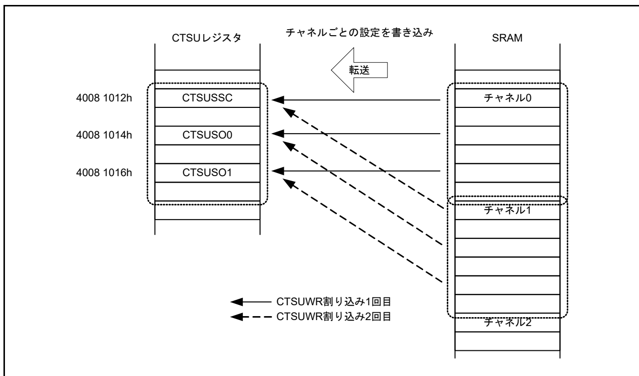
図 49.19 CTSU_CTSUWR 割り込みを用いた DTC 転送動作例
