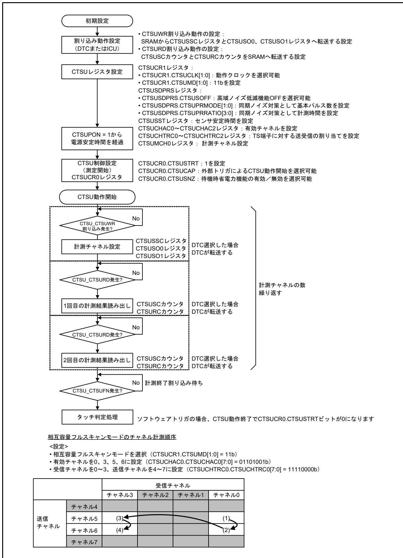
図 49.16 相互容量フルスキャンモードのソフトウェアフローと動作例
