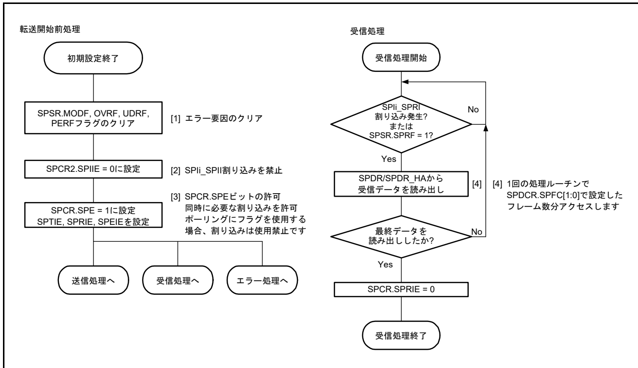
図 36.42 スレーブモードでの受信フロー
