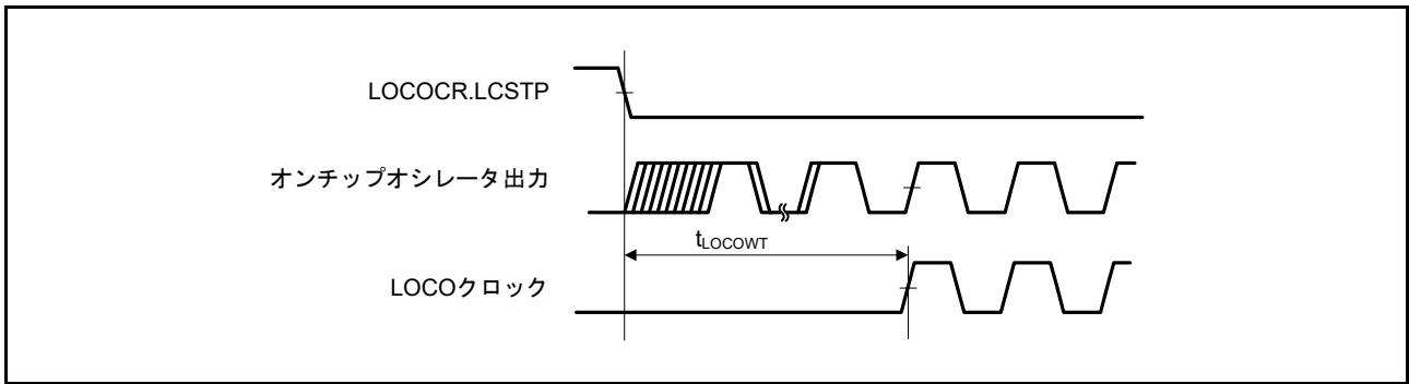
図 55.10 LOCO クロック発振開始タイミング
