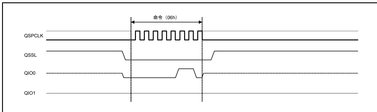
図 37.29 ライトイネーブルバスサイクル
