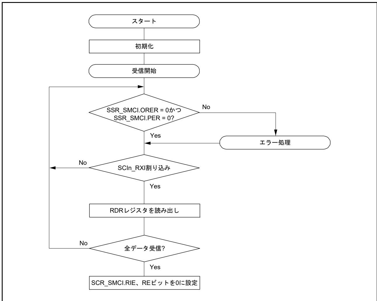
図 32.56 スマートカードインタフェース受信のフローチャート例
