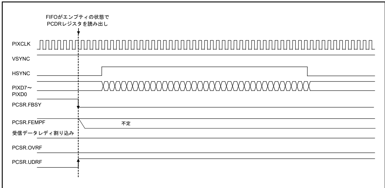
図 42.15 アンダーラン検出時の動作
