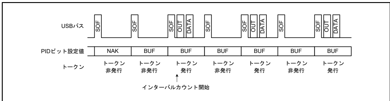
図 31.17 IITV = 1 の場合のトークン発行の有無
