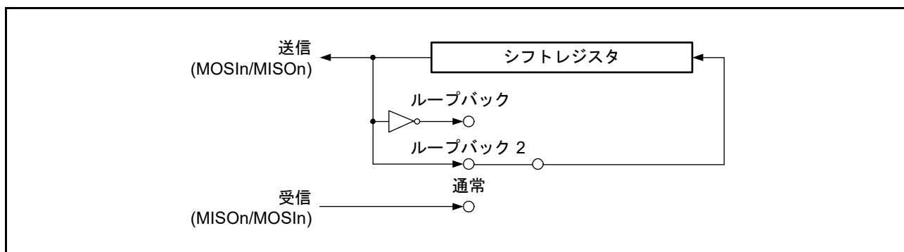
図 36.49 ループバックモード時のシフトレジスタ入出力経路の構成 (マスタモード)
