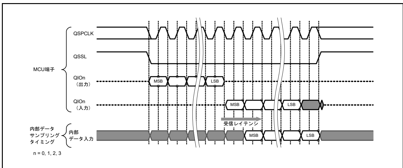
図 37.15 受信レイテンシ
