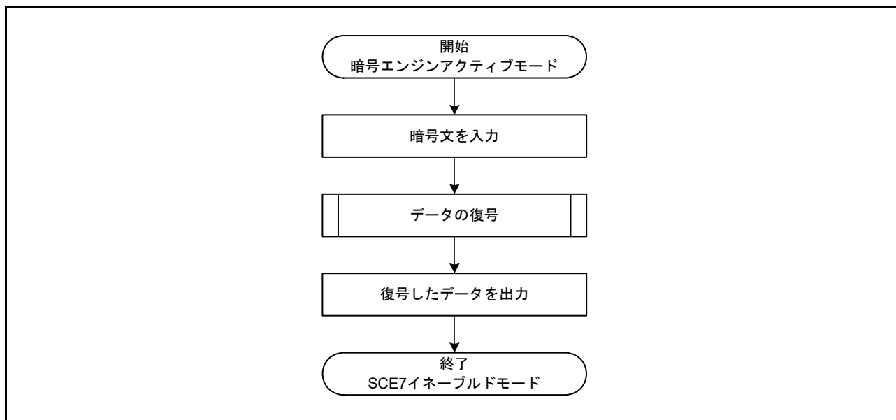
図 44.5 復号フローチャート
