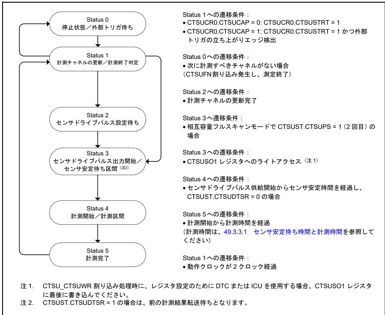
図 49.11 ステータス動作遷移図
