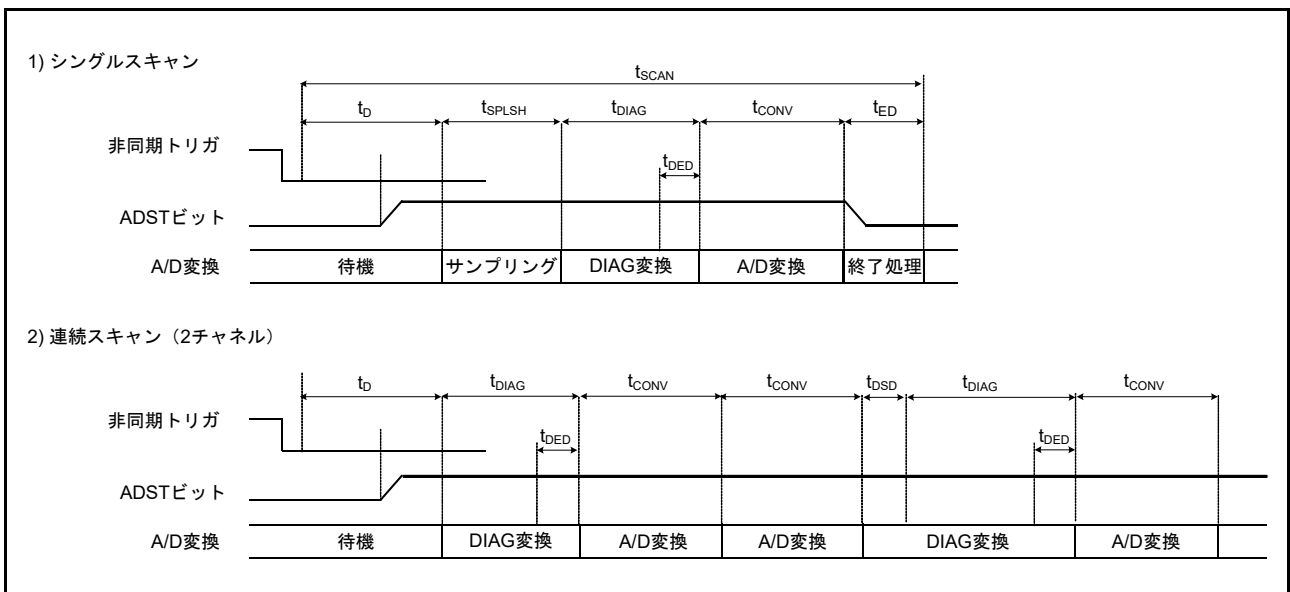
図 45.35 スキャン変換のタイミング (非同期トリガ入力 (ADTRG0) 起動の場合)
