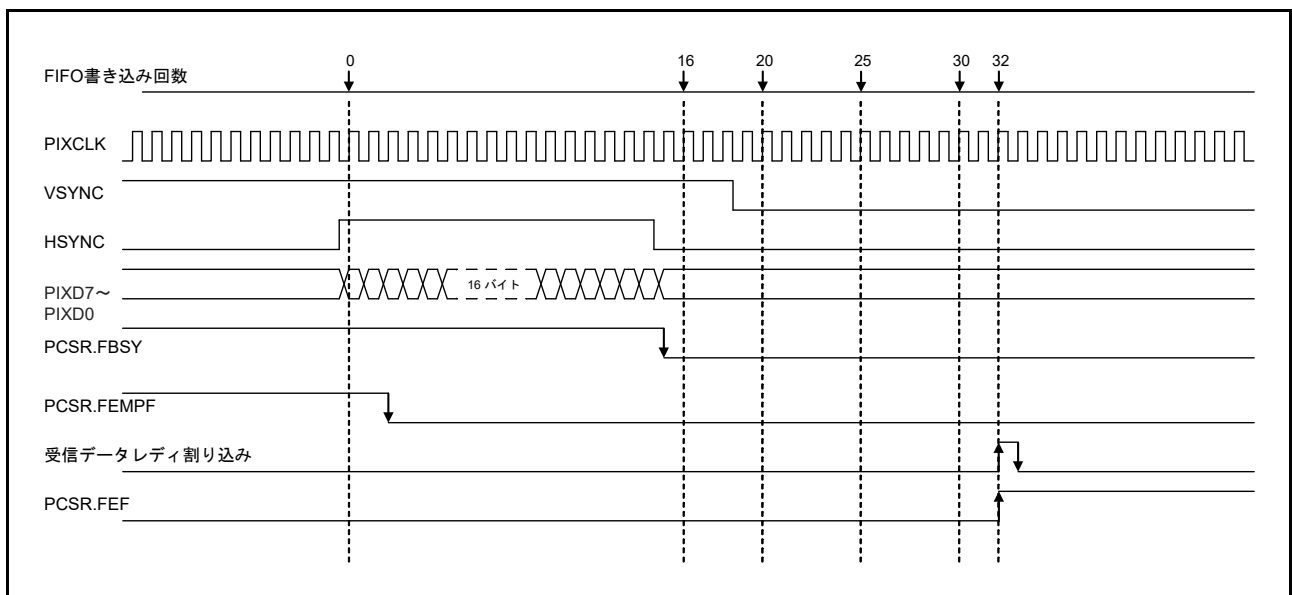
図 42.13 フレームエンドでの継続受信動作例
