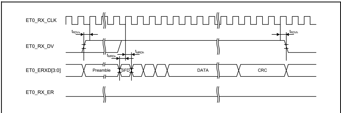
図 55.71 正常動作時の MII 受信タイミング
