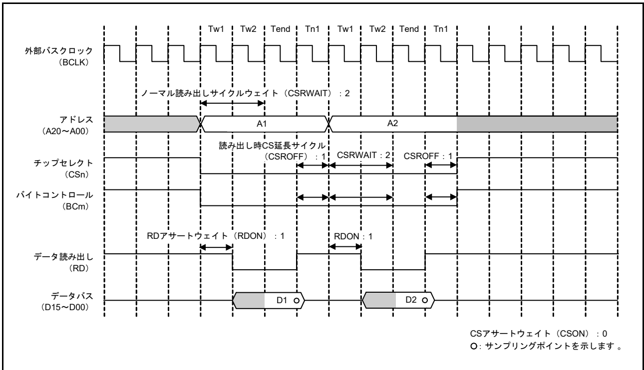
図 15.14 ノーマルリードアクセスの動作例 (1 転送要求に対して 2 回バスアクセスが発生する場合) (n = 0 ~ 7 および m = 0, 1)
