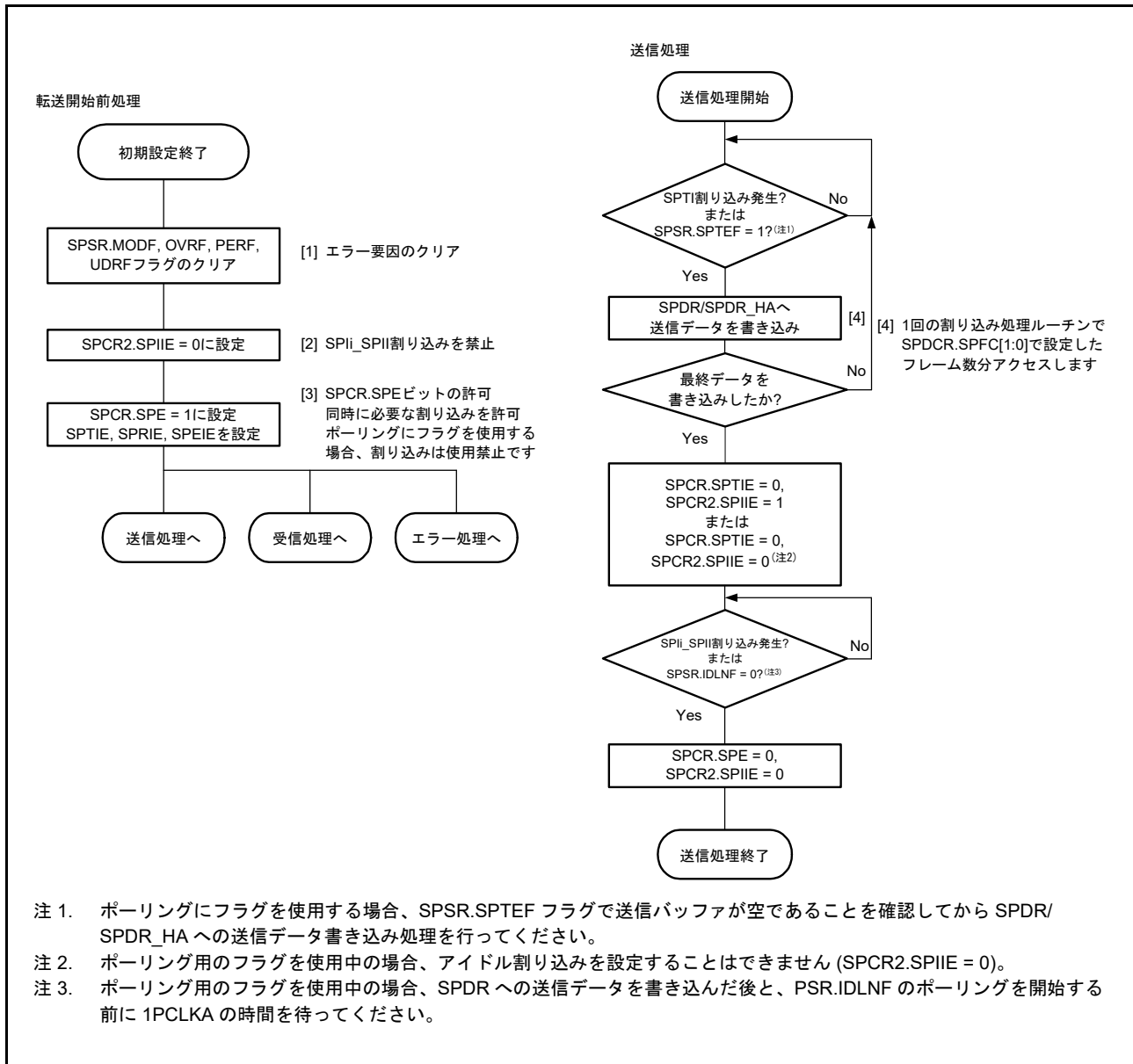
図 36.37 マスタモードでの送信フロー
