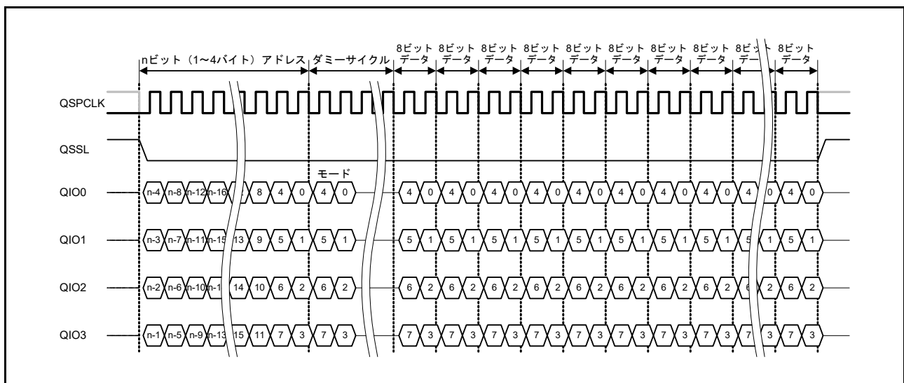
図 37.26 XIP モード時のファストリード Quad I/O バスサイクル
