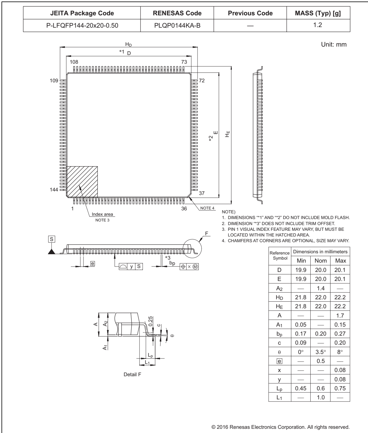
図 2.2 144 ピン LQFP
