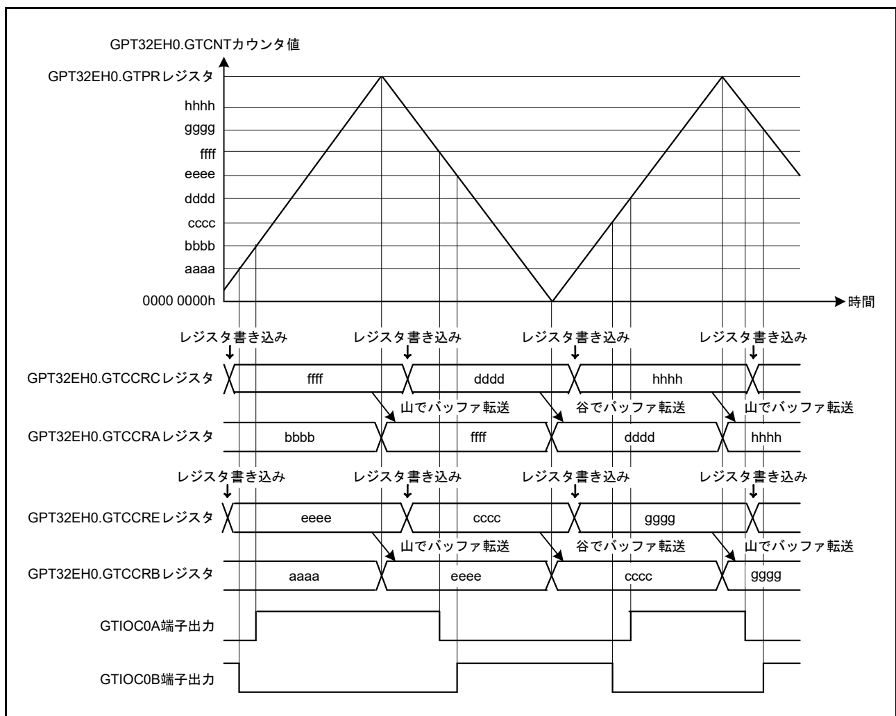
図 23.39 三角波 PWM モード 2 動作例 (バッファ動作、カウントスタート時 GTIOC0A 端子 = Low 出力 / GTIOC0B 端子 = High 出力、GTCCRA/GTCCRB レジスタのコンペアマッチでトグル出力、周期の終わりで出力保持の場合)
