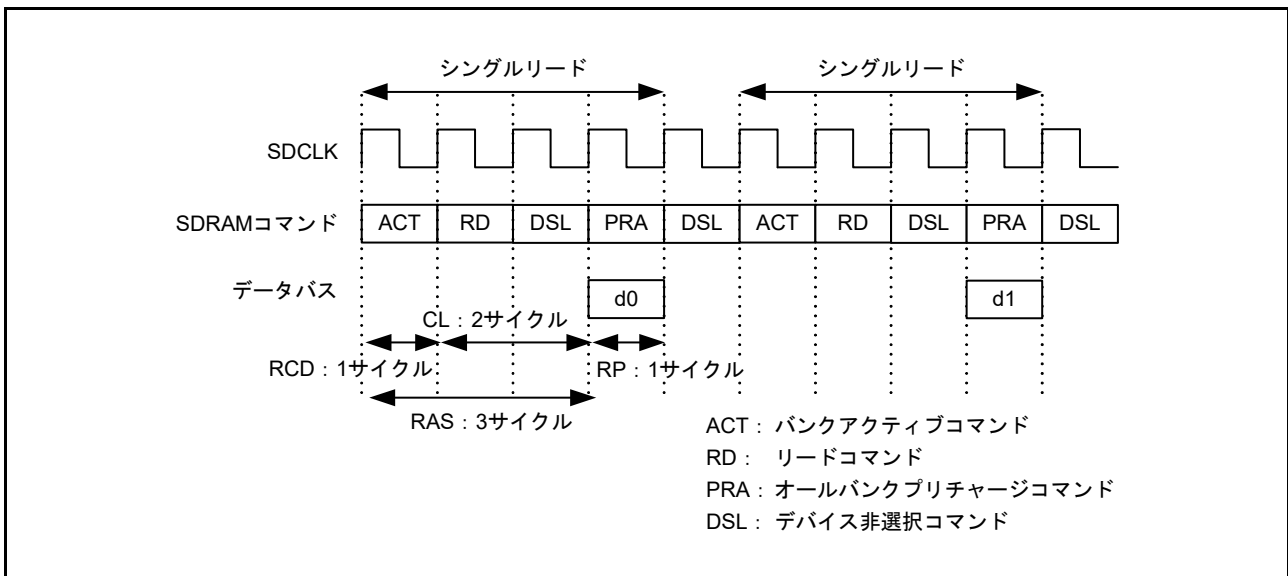
図 15.56 シングルリードタイミング例 (4)
