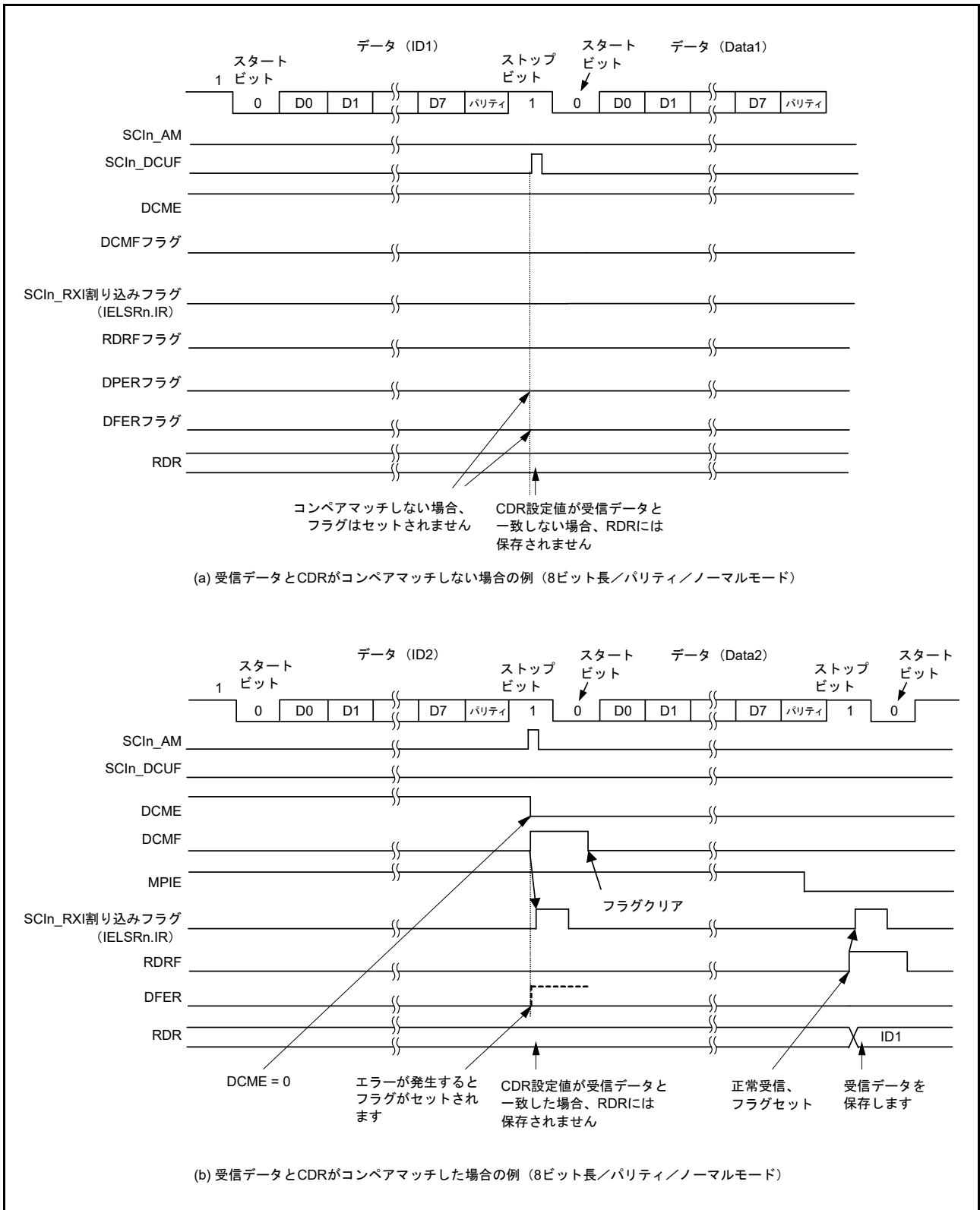
図 32.5 アドレス一致検出の例 (1) (通常モード)
