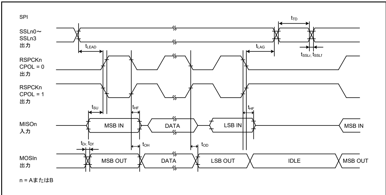
図 55.50 CPHA = 0 で、PCLKA/2 にピットレートが設定されている場合におけるマスタの SPI タイミング
