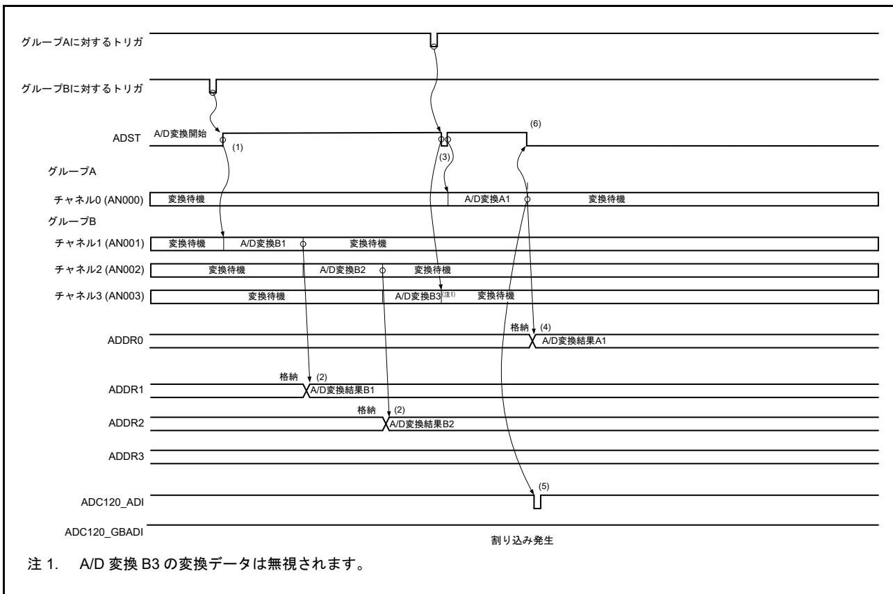
図 45.29 グループ A 優先制御の動作例 (4) (ADGSPCR.GBRSCN = 0、ADGSPCR.GBRP = 0 の場合)
