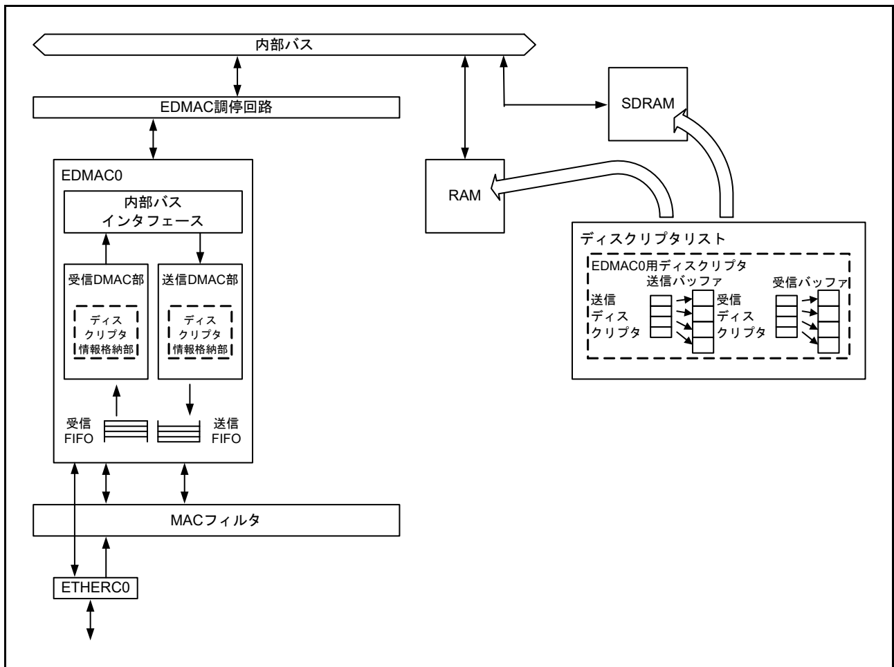
図 30.2 メモリ内のディスクリプタおよび送受信バッファの構成
