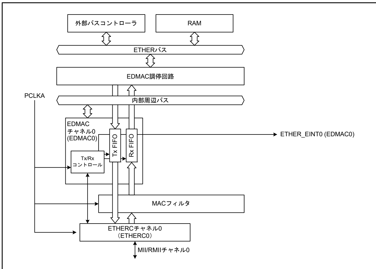
図 30.1 EDMAC の構成
