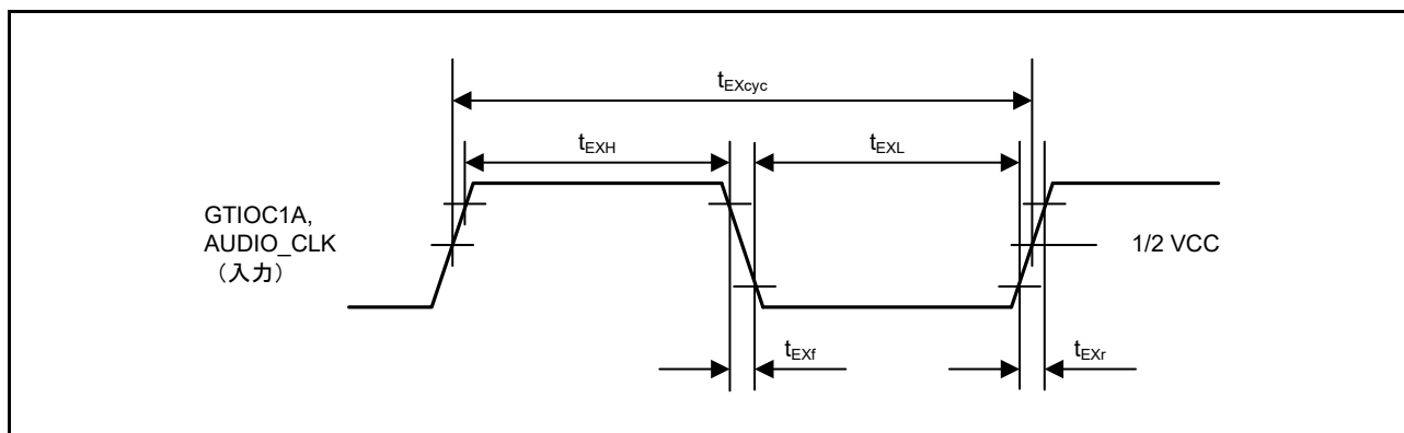
図 55.59 クロック入力タイミング
