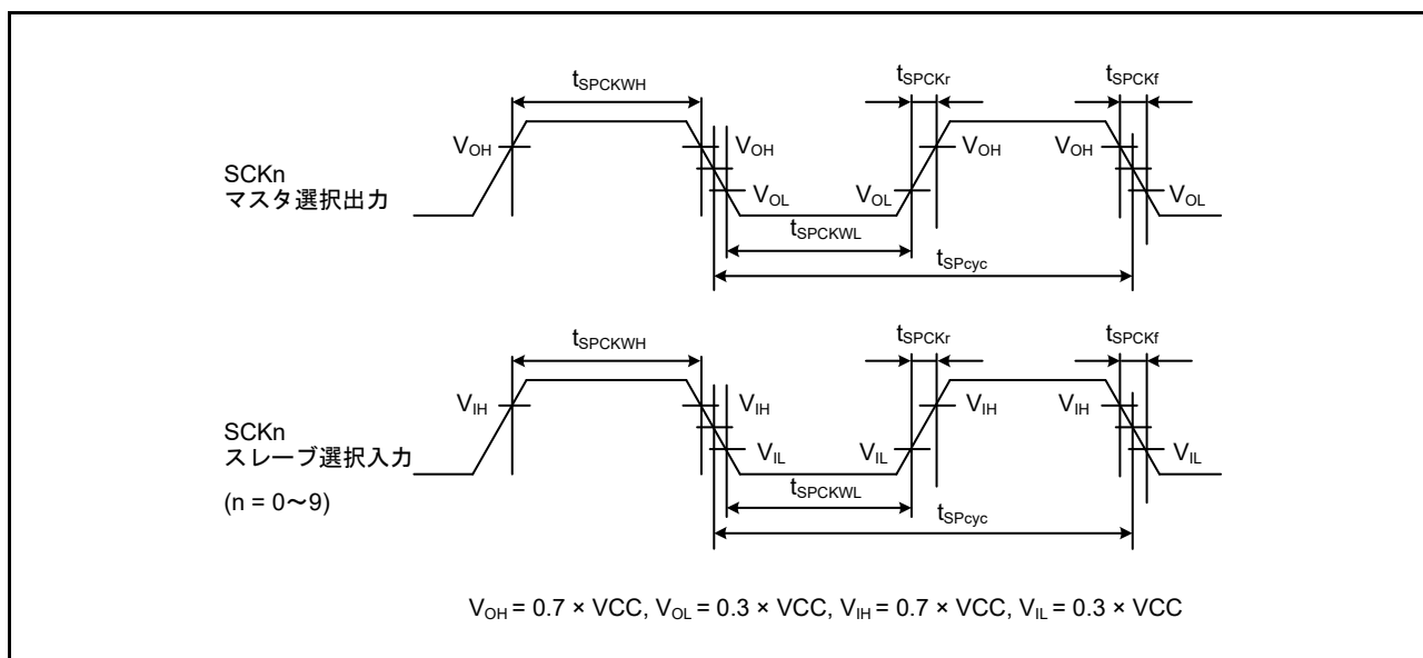
図 55.42 SCI 簡易 SPI モードクロックタイミング
