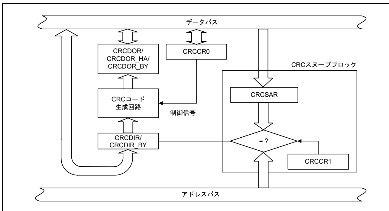
図 38.1 CRC のブロック図
