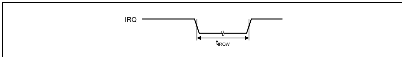
図 55.19 IRQ 割り込み入力タイミング
