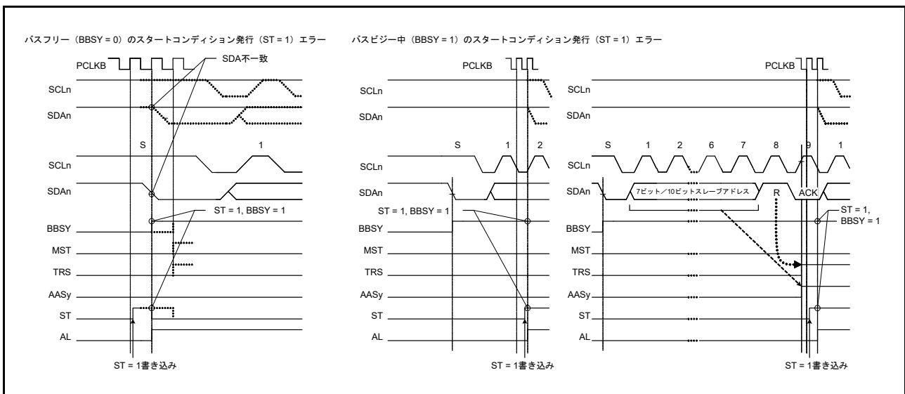
図 34.42 スタートコンディション発行時のアービトレーションロスト (MALE = 1 の場合)
