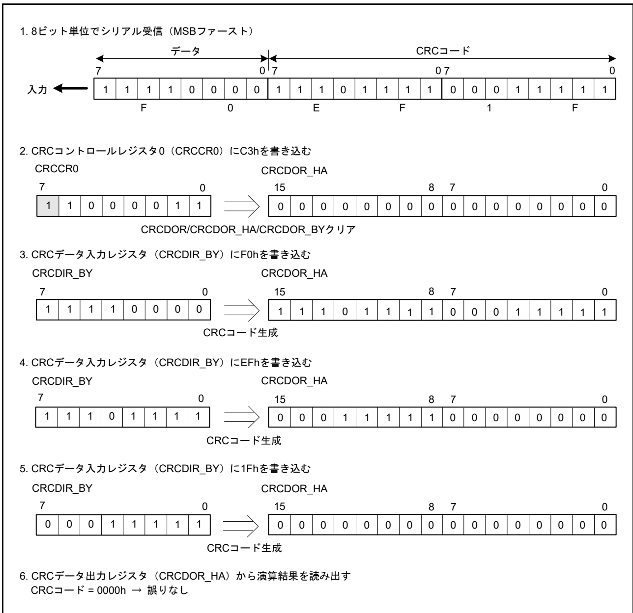
図 38.5 MSB ファーストのデータ受信
