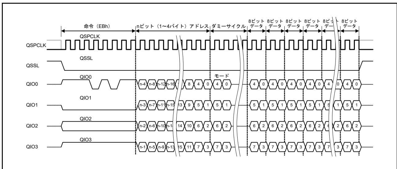
図 37.25 ファストリード Quad I/O バスサイクル
