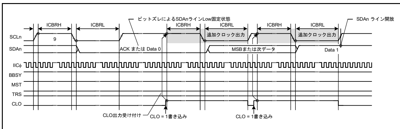
図 34.49 SCL クロック追加出力機能 (CLO ビットの使用)
