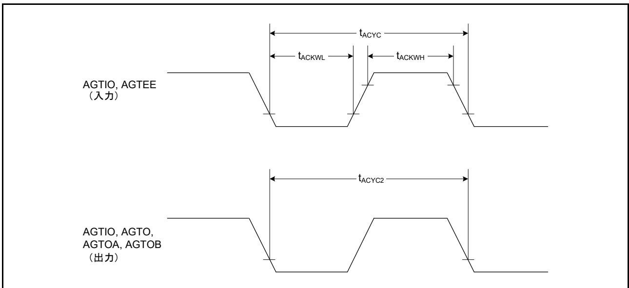
図 55.37 AGT 入出力タイミング
