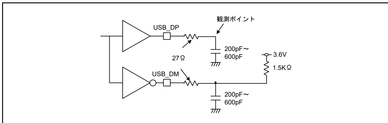
図 55.78 Low-speed モードにおける測定回路
