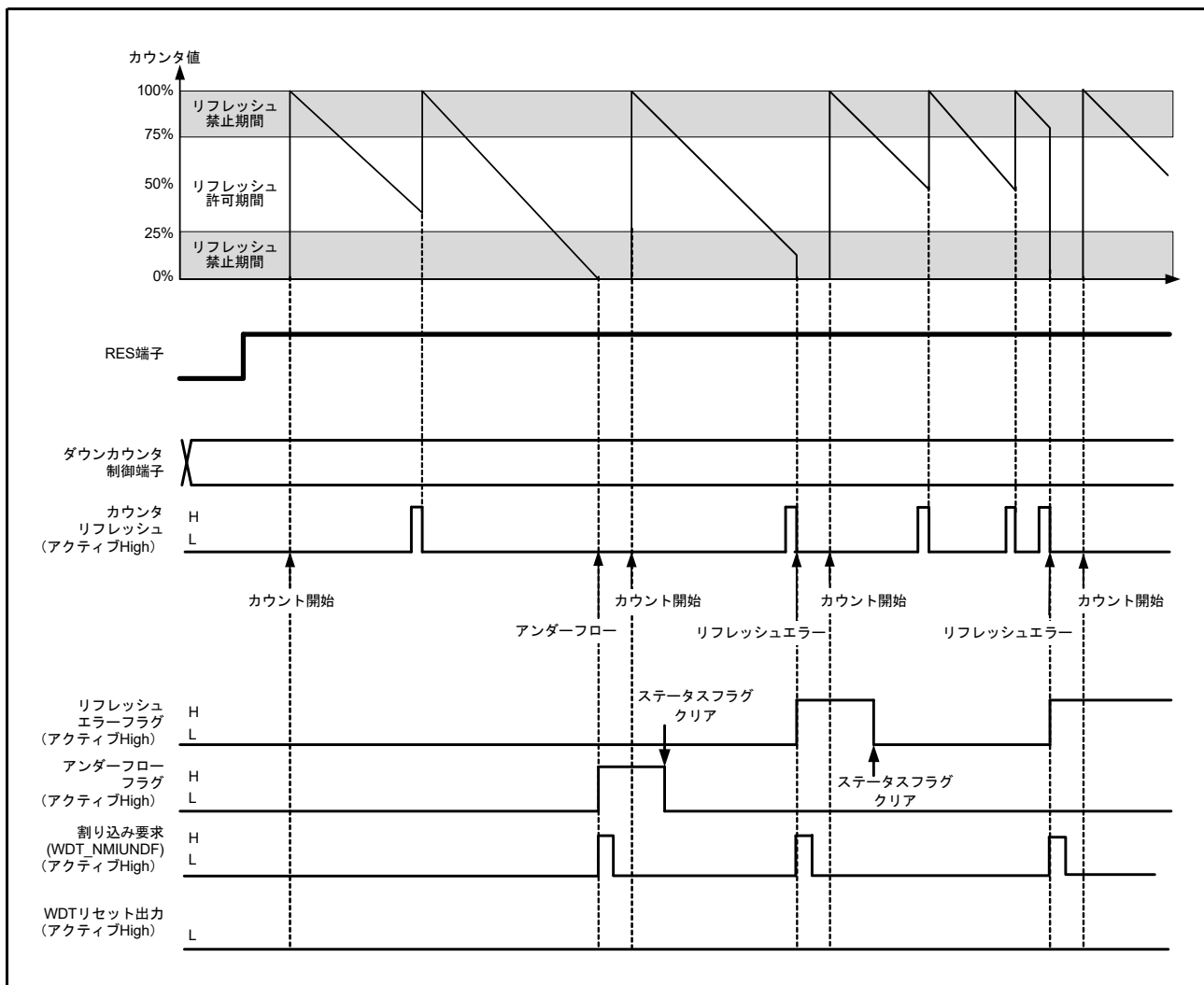
図 27.4 オートスタートモードでの動作例
