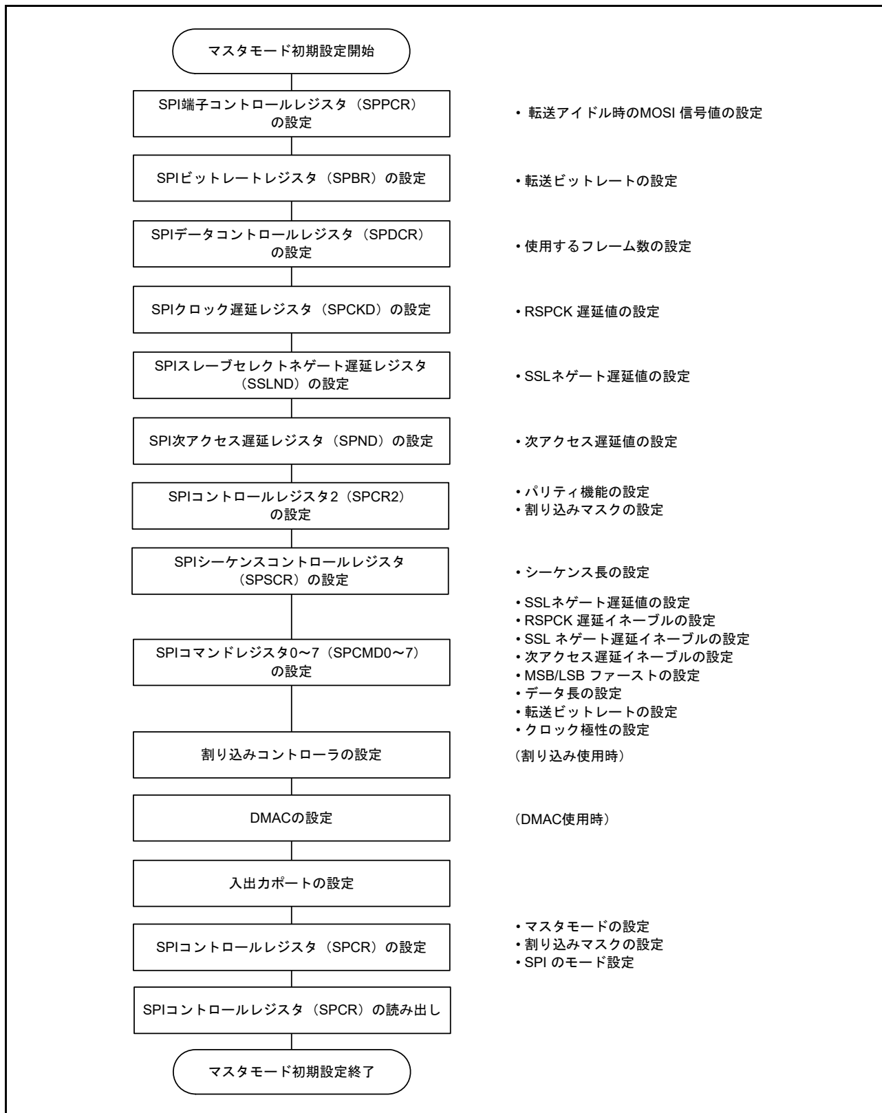
図 36.47 マスタモード時のクロック同期式動作の初期化フロー例
