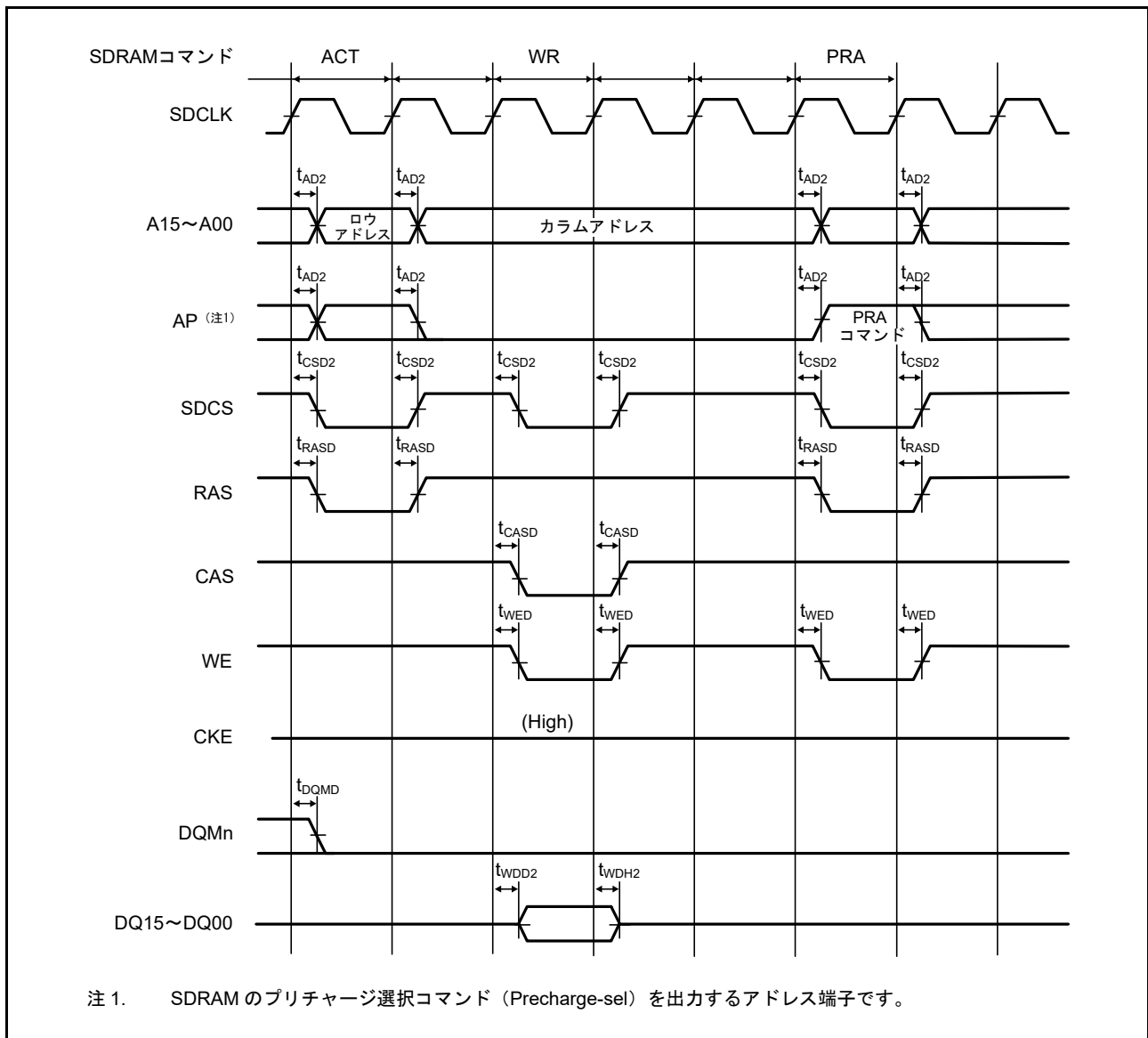
図 55.28 SDRAM シングルライトタイミング
