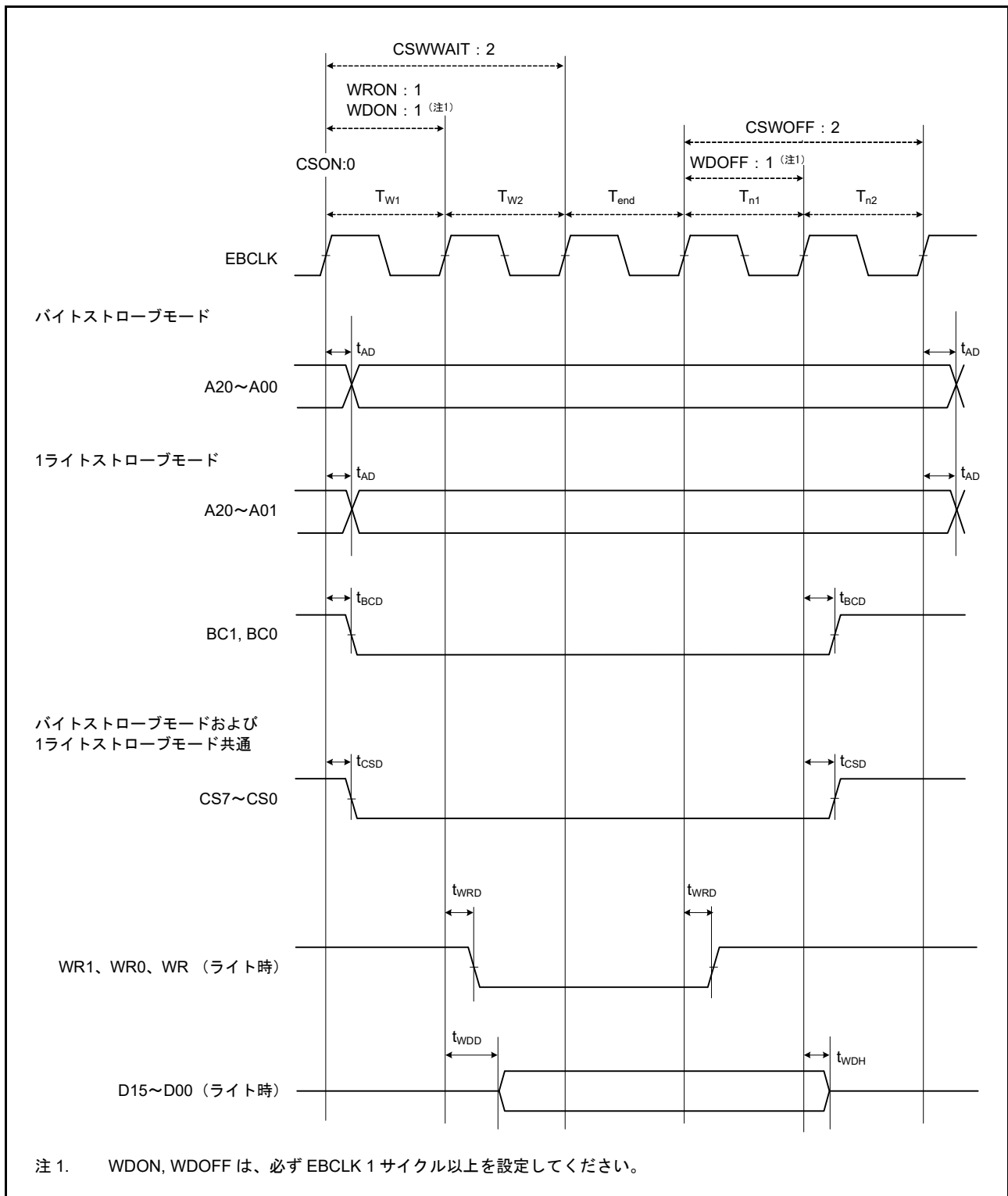
図 55.23 バスクロック同期を使用したノーマルライトサイクルの外部バスタイミング
