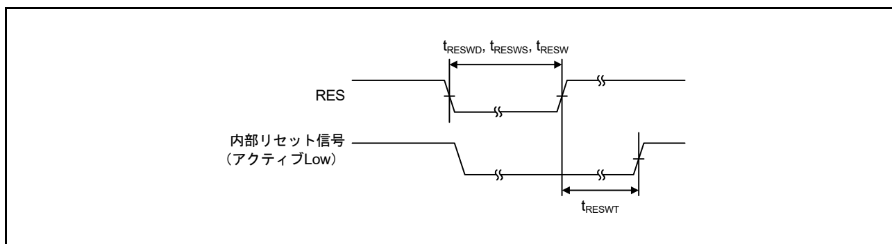
図 55.14 リセット入力タイミング
