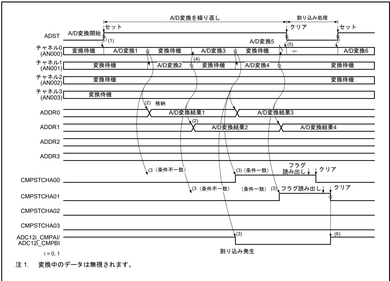
図 45.31 コンペア機能の動作例 (AN000 ~ AN003 を比較)
