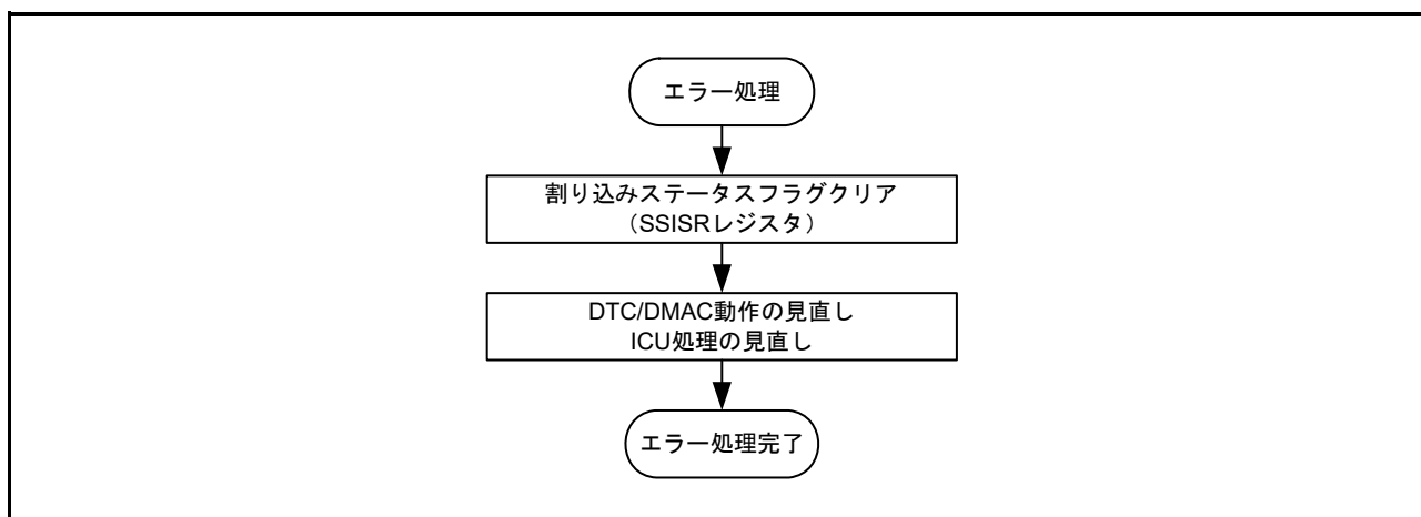
図 39.57 エラー処理手順
