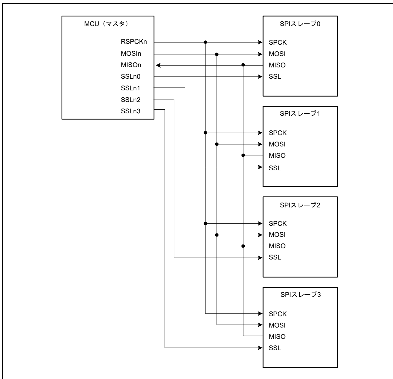
図 36.8 シングルマスタ/マルチスレーブの構成例 (MCU はマスタ)
