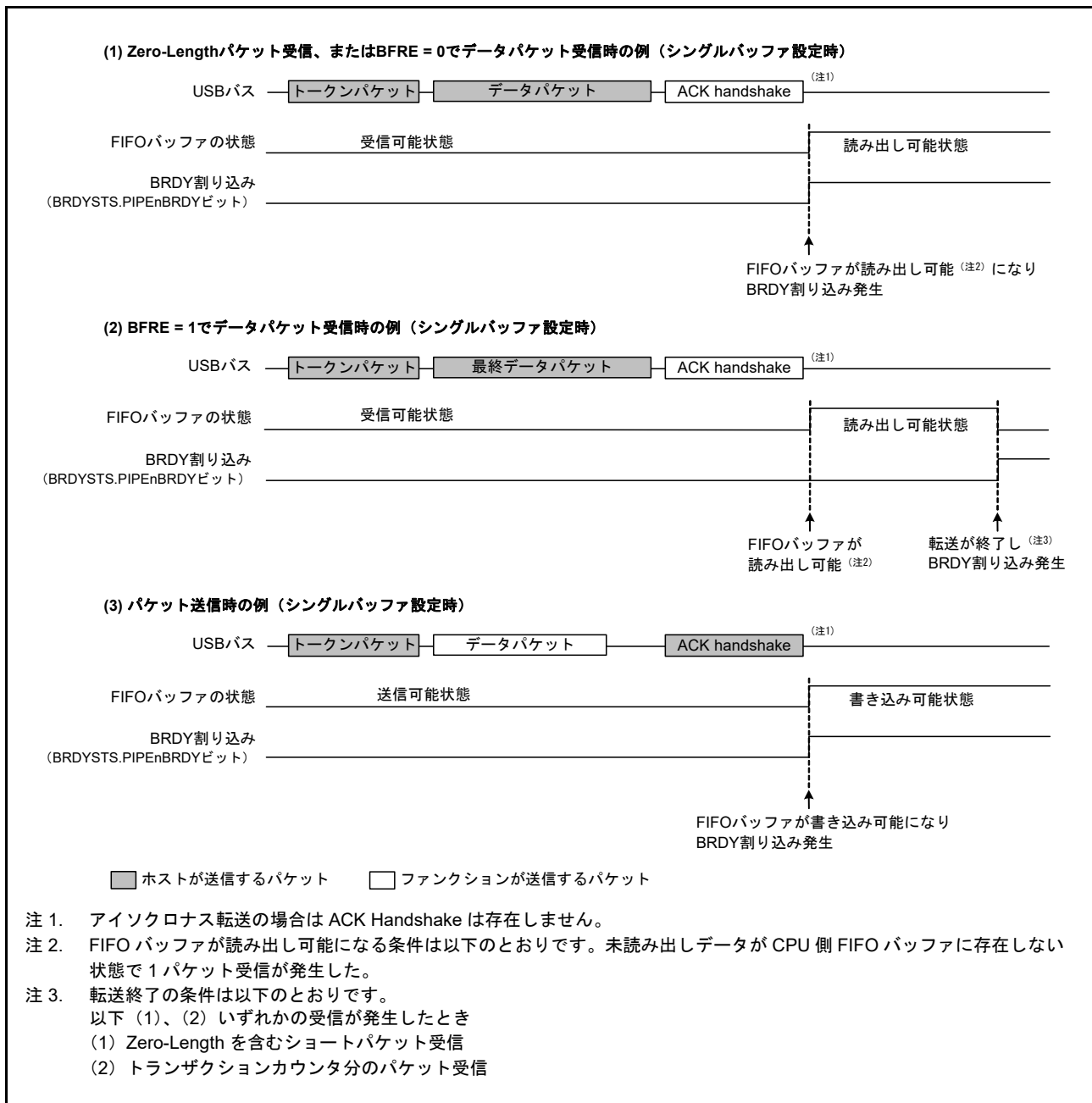
図 31.11 BRDY 割り込み発生タイミング
