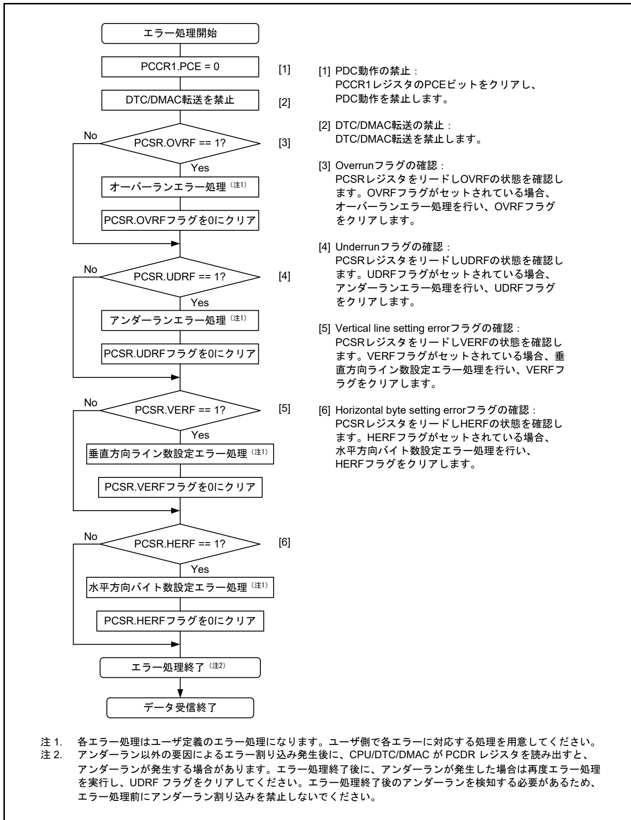
図 42.20 エラー処理フロー例
