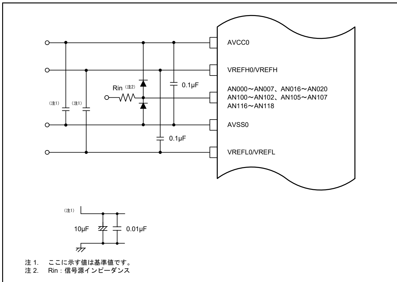
図 45.41 アナログ入力用保護回路例
