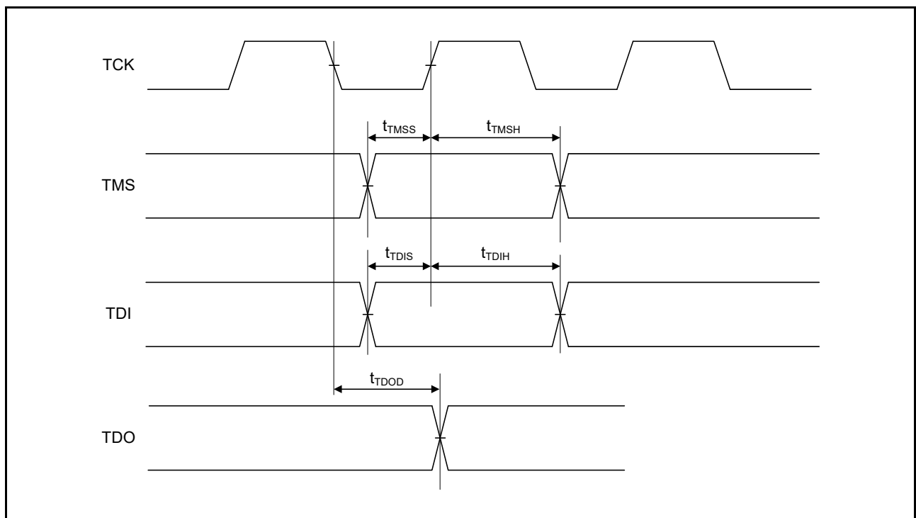
図 55.93 JTAG 入出力タイミング
