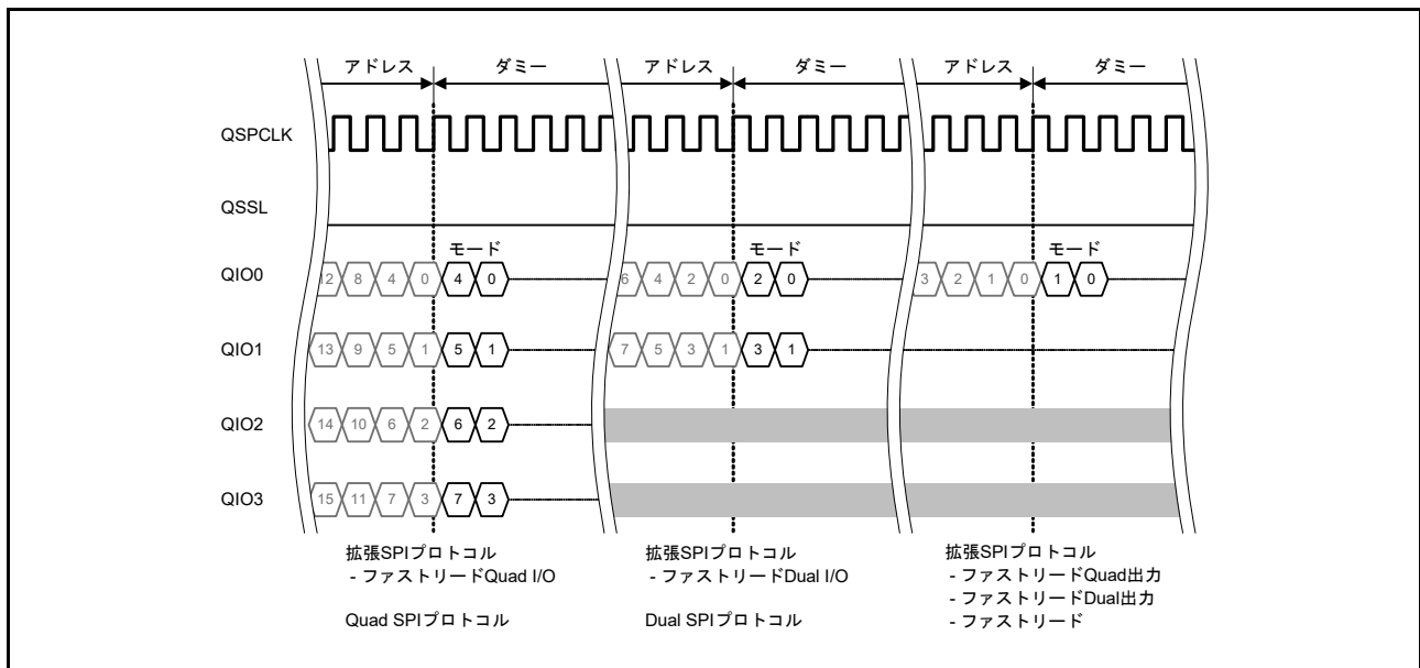
図 37.33 XIP モード制御データ
