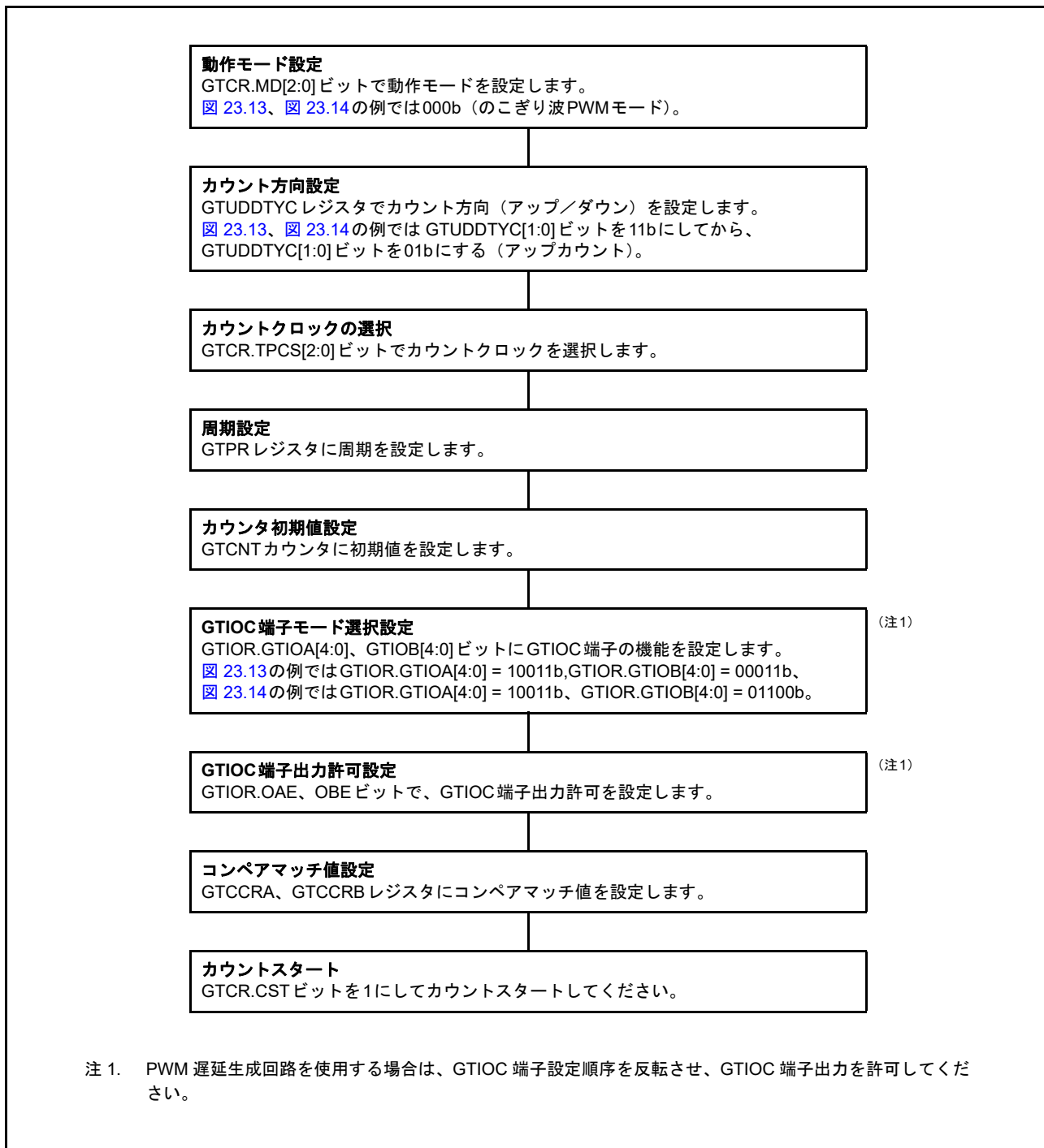
図 23.15 トグル出力動作設定例
