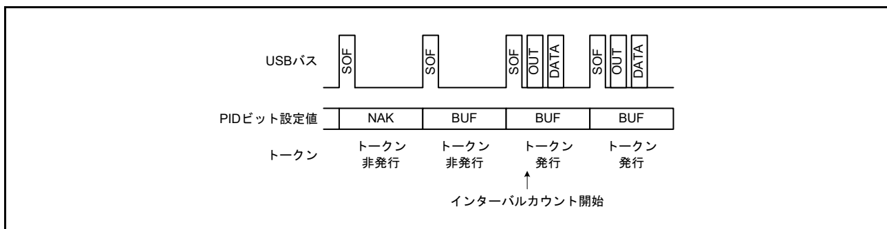
図 31.16 IITV = 0 の場合のトークン発行の有無
