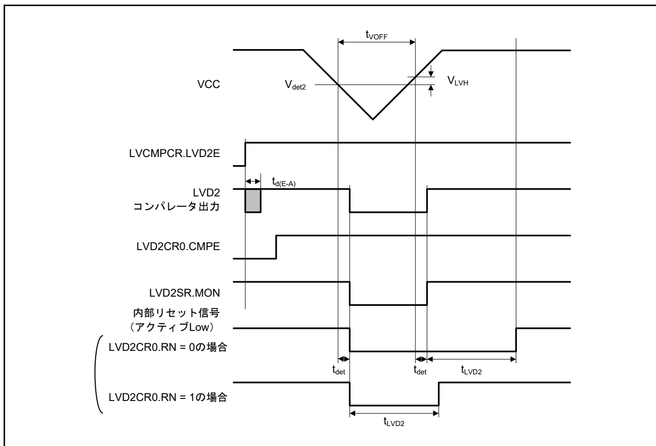
図 55.86 電圧検出回路タイミング ( V_{det2} )
