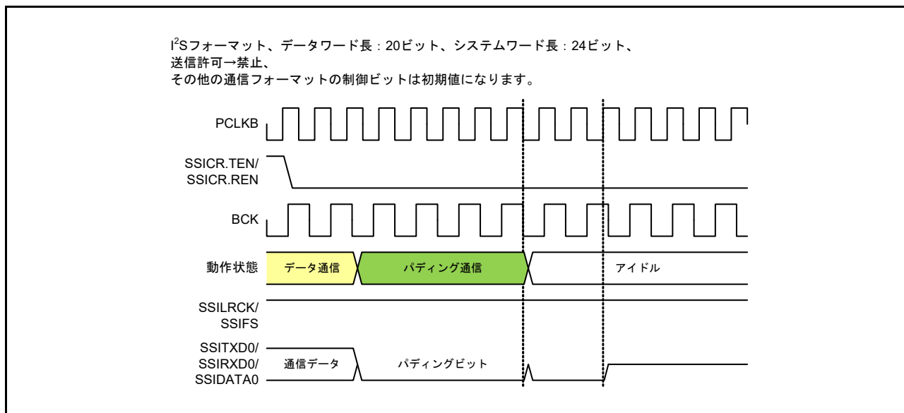
図 39.51 パディング通信からの停止
