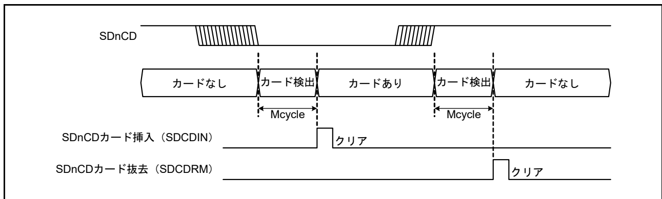
図 41.7 SDnCD によるカード検出例
