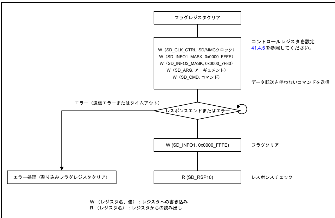
図 41.10 データがないコマンドのフロー例
