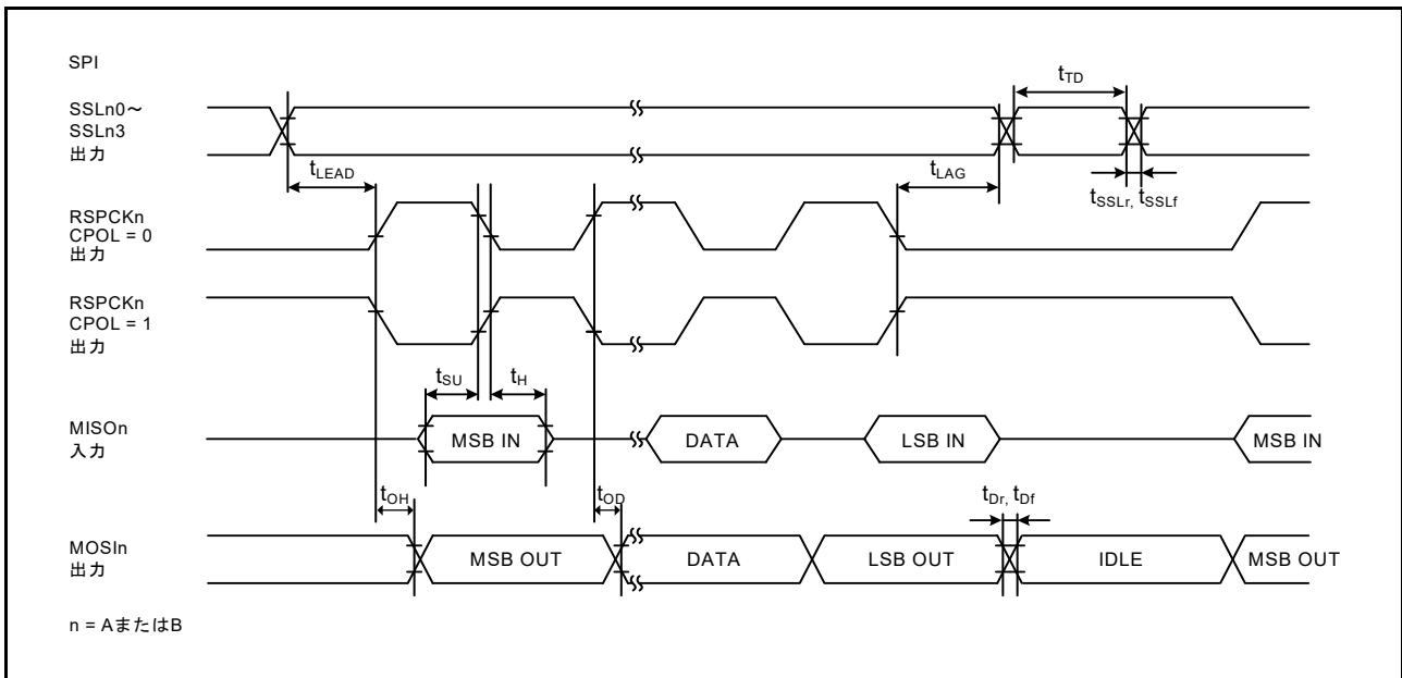
図 55.51 CPHA = 1 の場合におけるマスタの SPI タイミング
