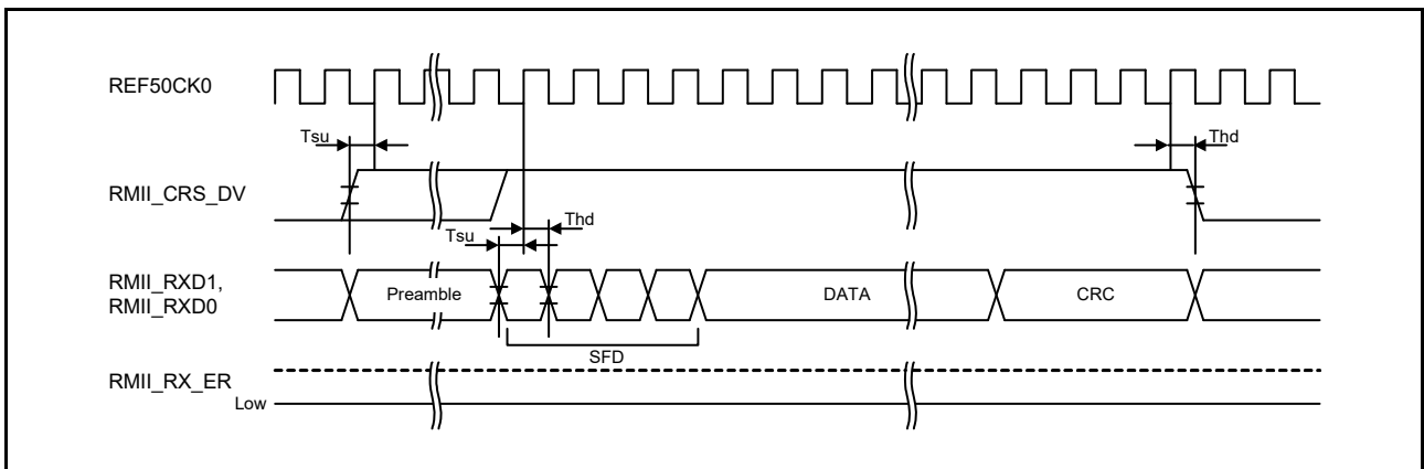
図 55.66 正常動作時の RMII 受信タイミング
