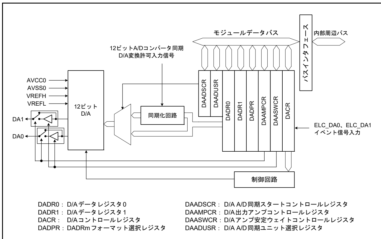
図 46.1 DAC12のブロック図
