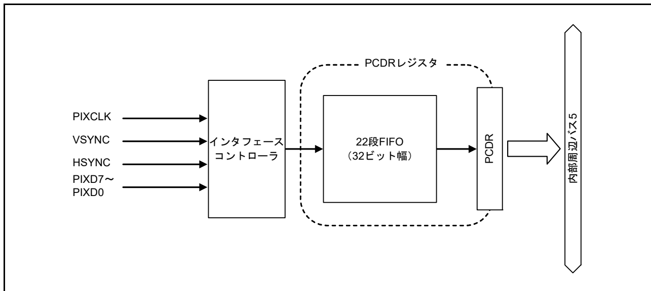
図 42.2 PCDR レジスタの構造図
