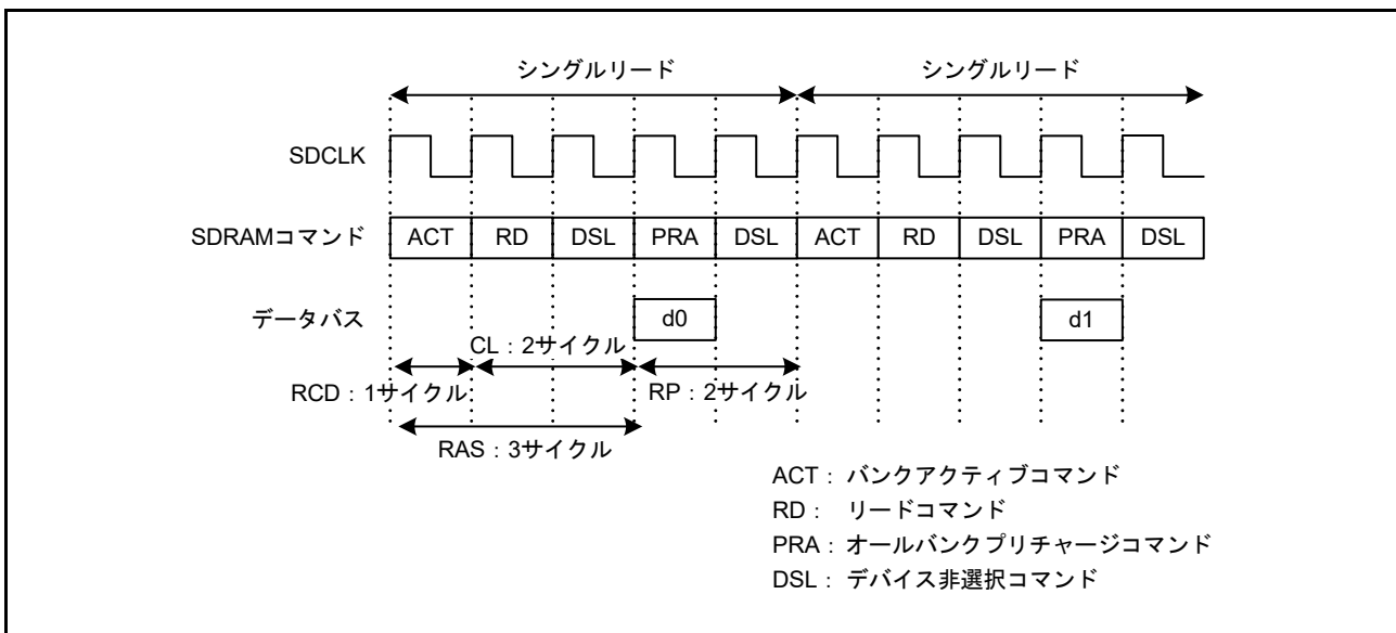
図 15.53 シングルリードタイミング例 (1)
