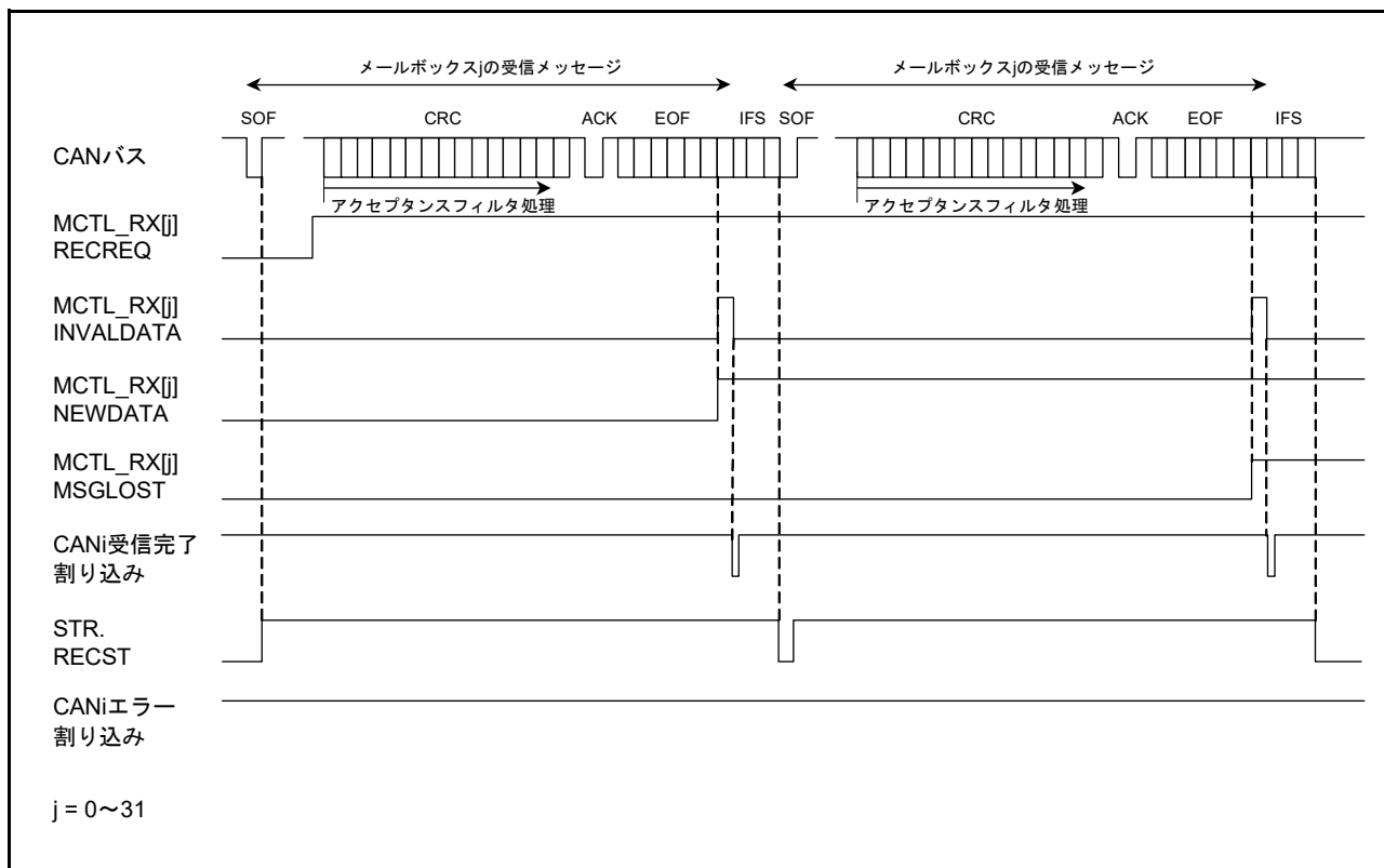
図 35.18 データフレーム受信時の動作例（オーバーライトモードの場合）
