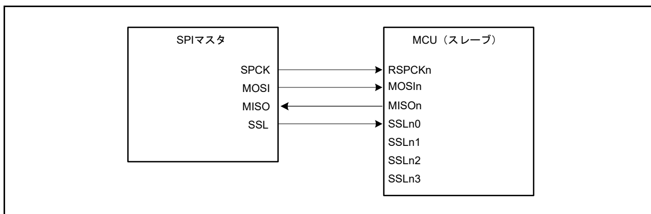
図 36.6 シングルマスタ/シングルスレーブの構成例 (MCU はスレーブ、CPHA = 0)
