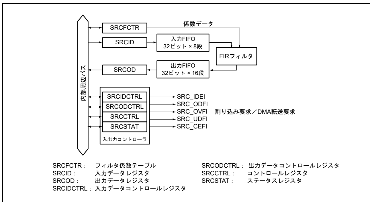
図 40.1 SRC のブロック図
