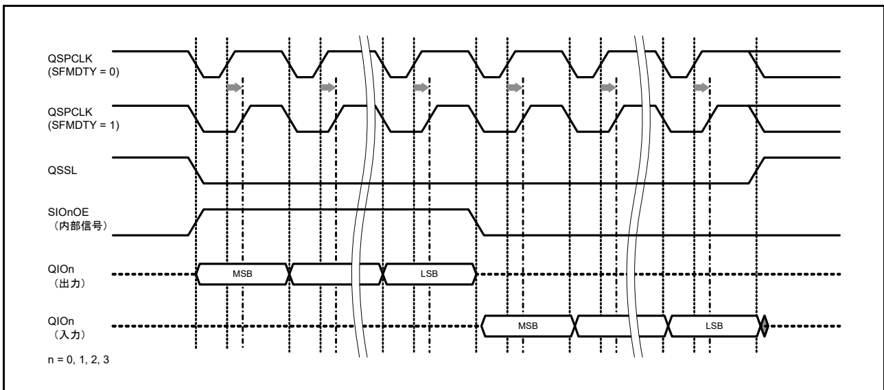
図 37.9 SFMMDTY ビットを使用した QSPCLK 信号デューティ比の補正例 (PCLKA を 3 通倍した場合)
