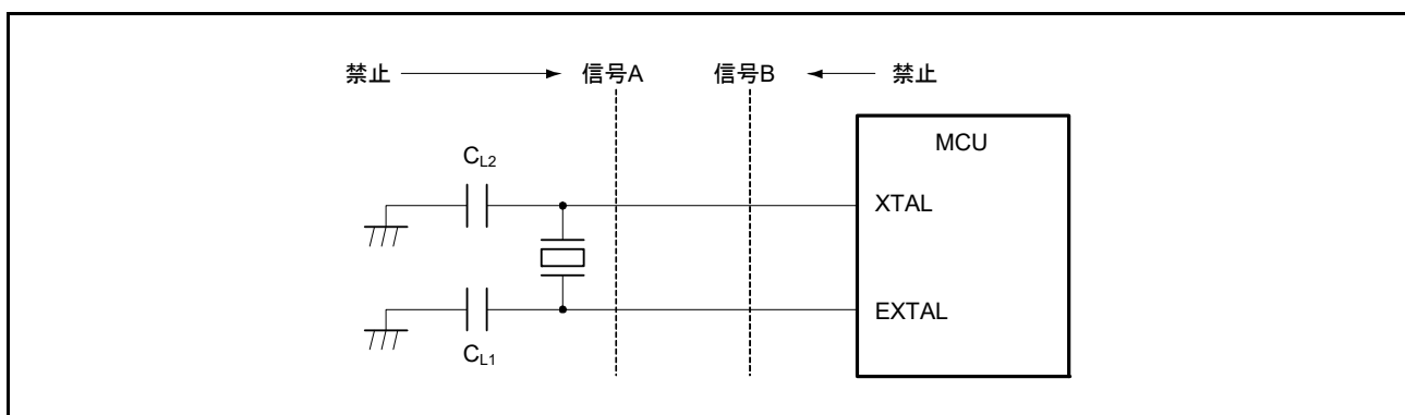
図 9.13 発振回路部のボード設計に関する注意事項 (メインクロック発振器の場合、サブクロック発振器も同様)
