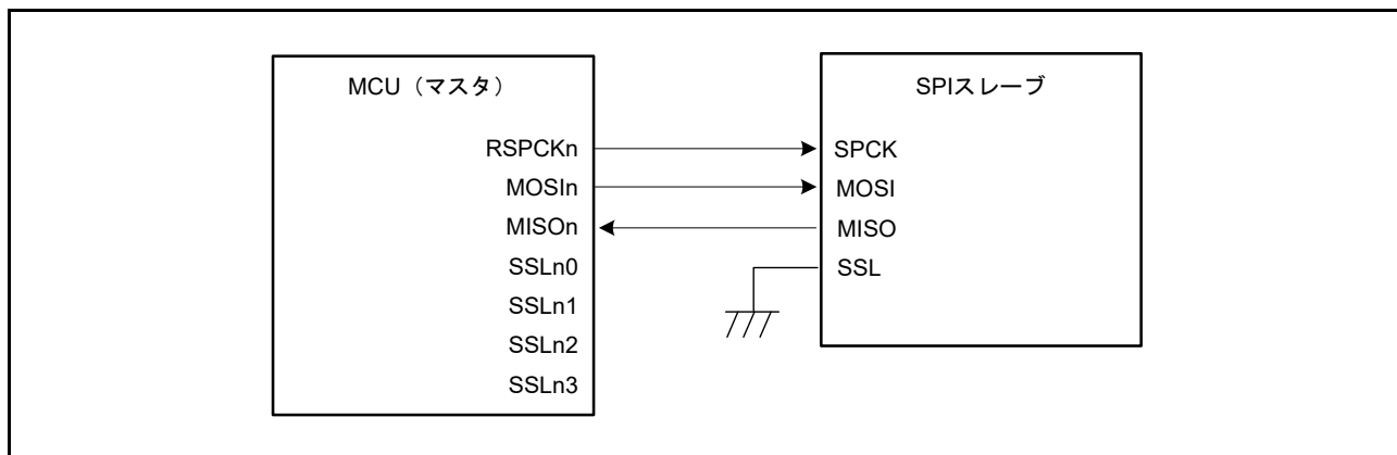
図 36.5 シングルマスタ/シングルスレーブの構成例 (MCU はマスタ)
