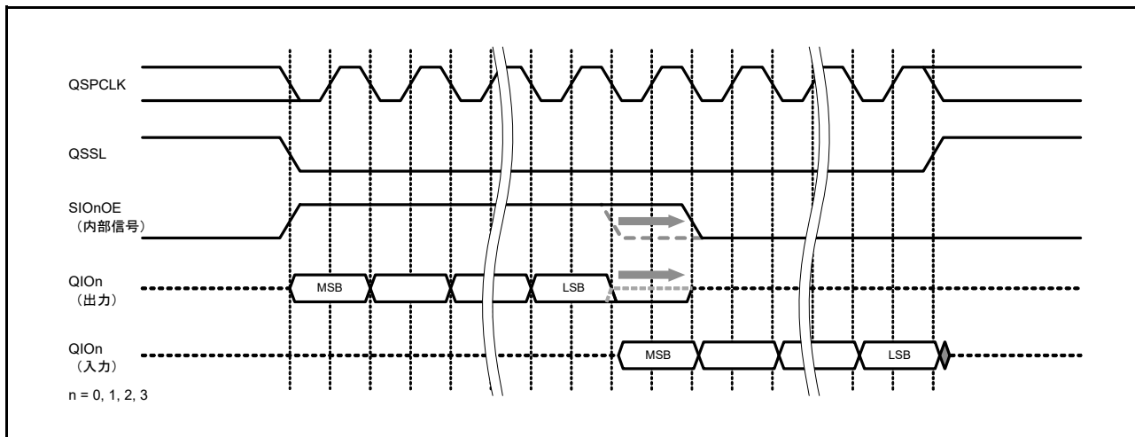
図 37.12 SFMOEX ビットを使用した出力許可ホールド時間調整
