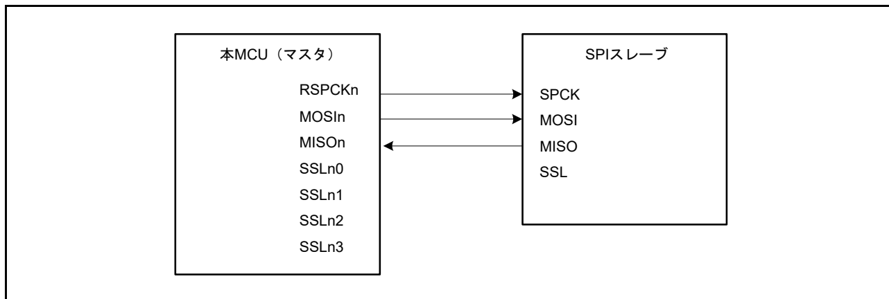
図 36.11 クロック同期式動作のマスター/スレーブの構成例 (MCU はマスター)
