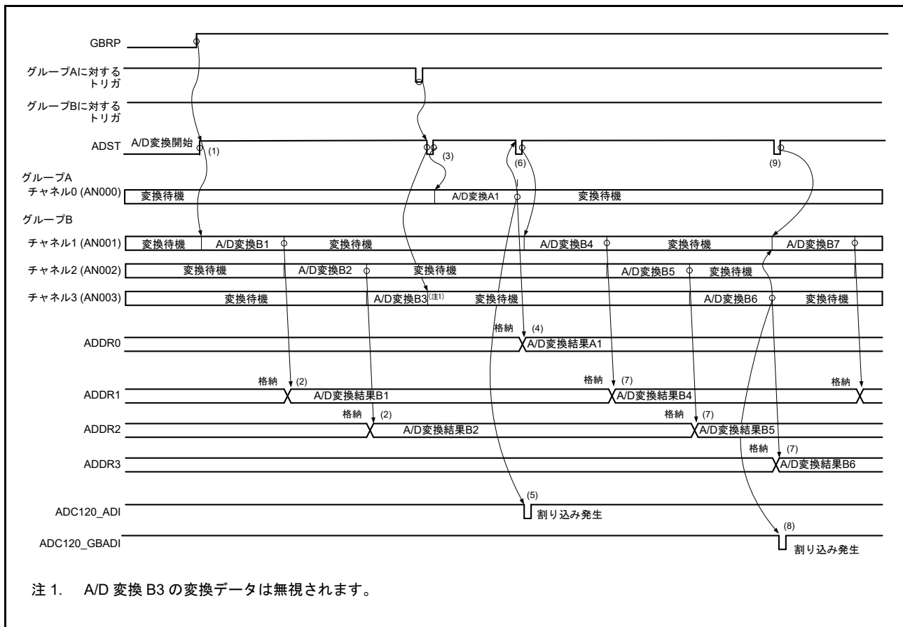
図 45.30 グループ A 優先制御の動作例 (5) (ADGSPCR.GBRP = 1 の場合)
