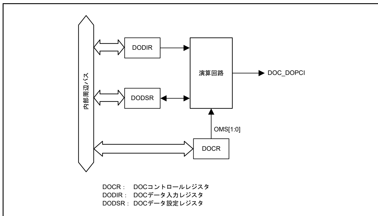
図 50.1 DOC ブロック図
