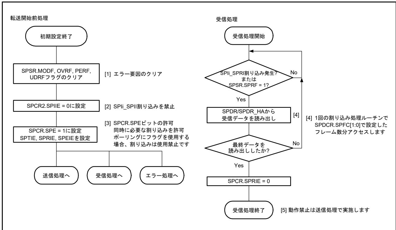
図 36.38 マスタモードでの受信フロー
