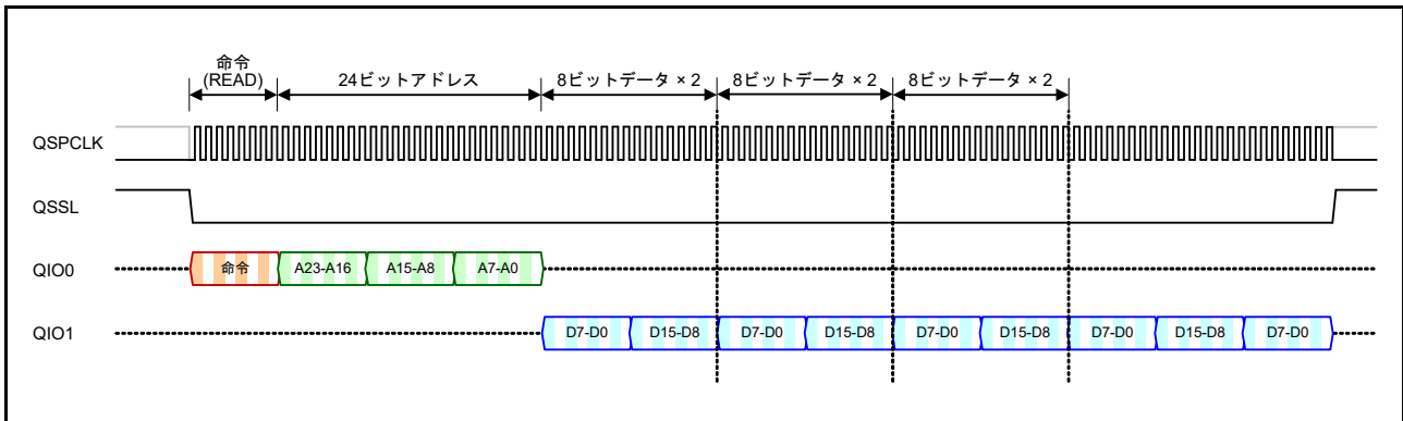
図 37.31 プリフェッチ機能を使用した連続データのリード動作
