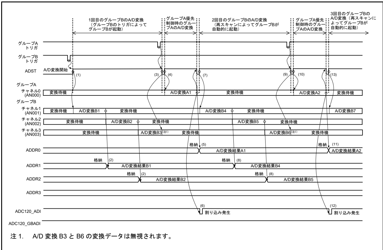
図 45.27 グループ A 優先制御の動作例 (2) (ADGSPCR.GBRSCN = 1、ADGSPCR.GBRP = 0 の場合)
