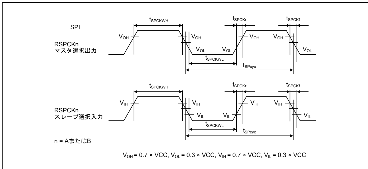
図 55.48 SPI クロックタイミング
