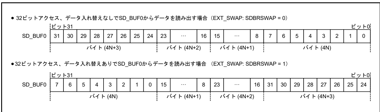
図 41.6 SD_BUF0 からの読み出し
