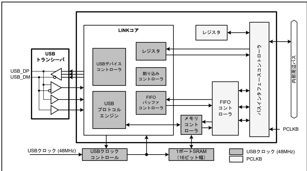
図 31.1 USBFS のブロック図
