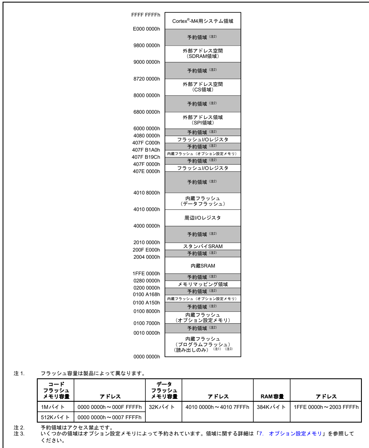
図 4.1 メモリマップ
