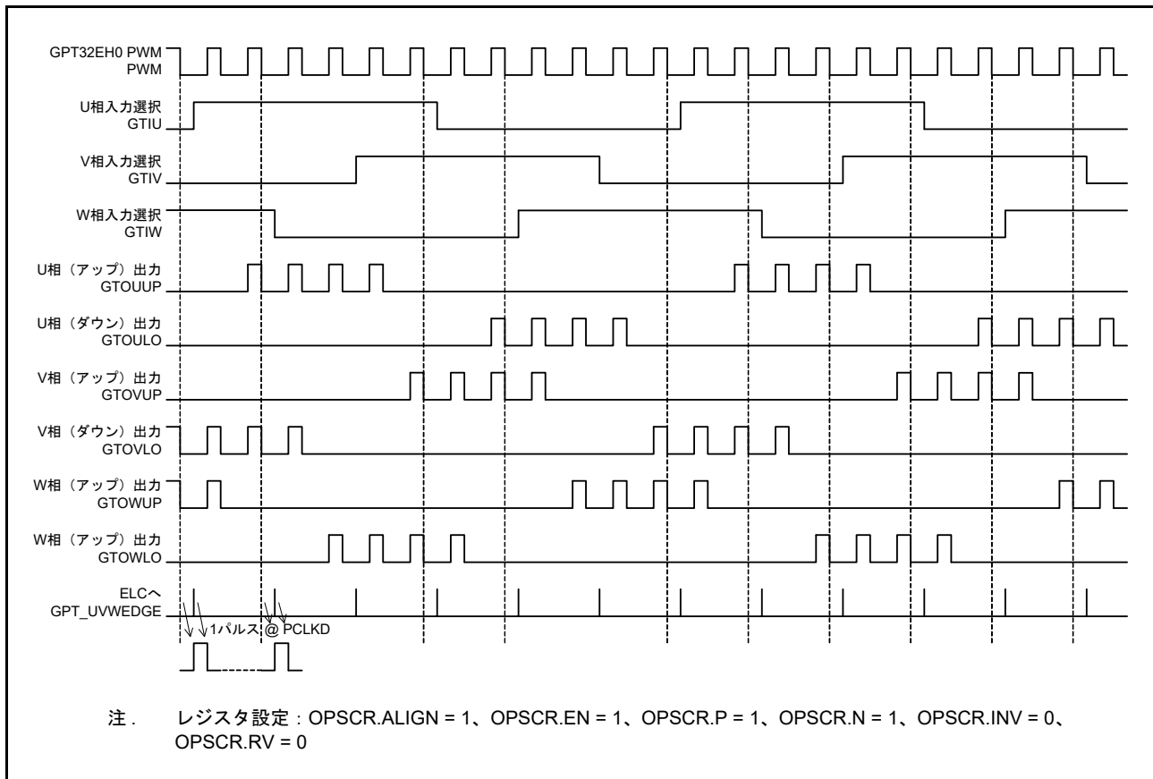
図 23.83 6 相 PWM 出力動作例 (チョップパ制御)
