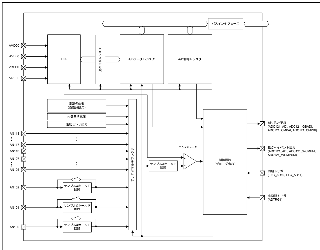
図 45.2 ADC12 (ユニット1) のブロック図
