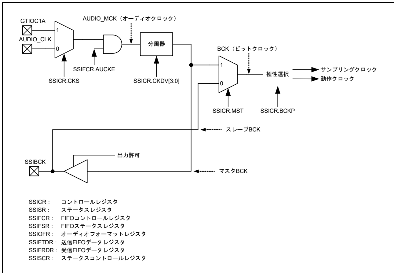
図 39.4 SSIE クロック構成
