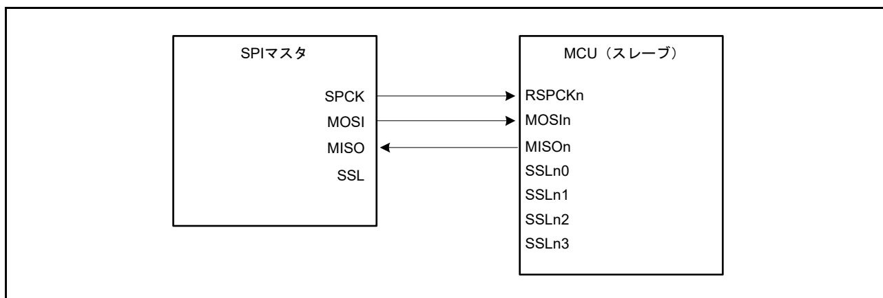
図 36.12 クロック同期式動作のマスター/スレーブの構成例 (MCU はスレーブ、CPHA = 1)
