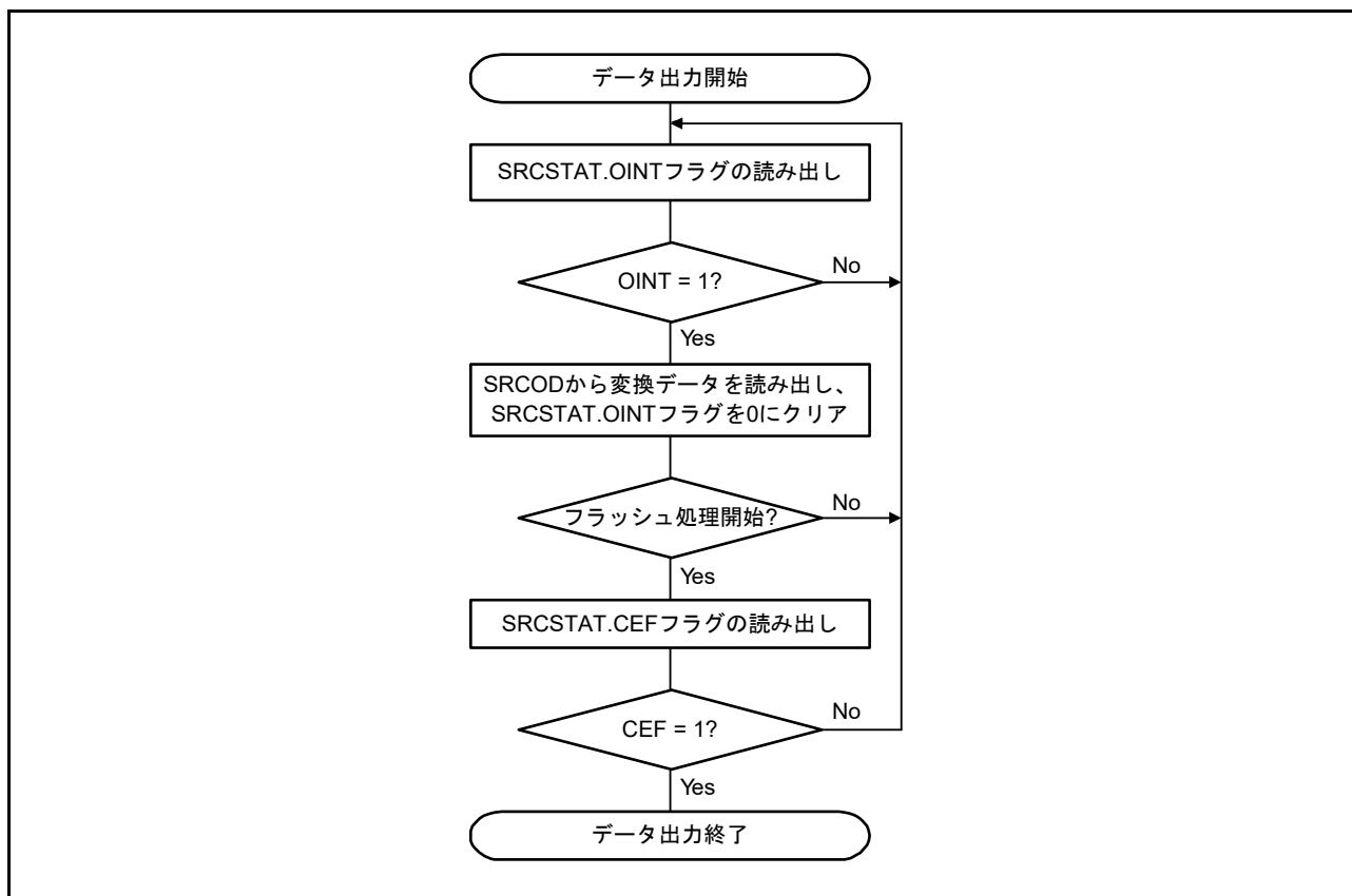
図 40.4 データ出力フロー
