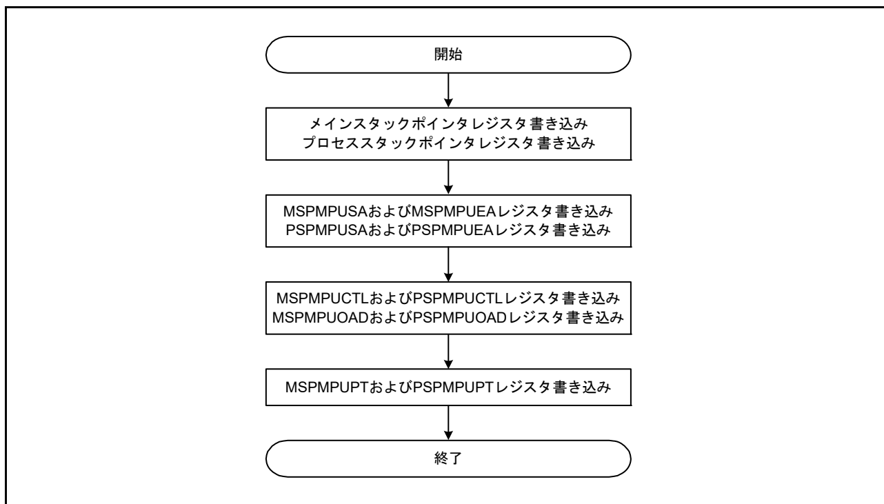
図 16.2 レジスタ設定フロー
