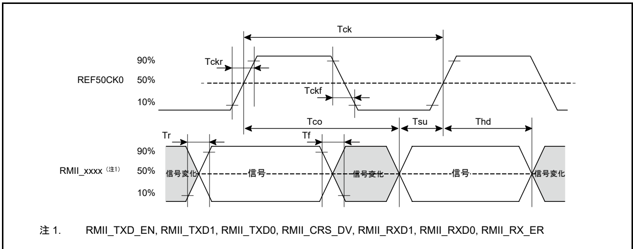
図 55.64 REF50CK0、RMII の信号タイミング
