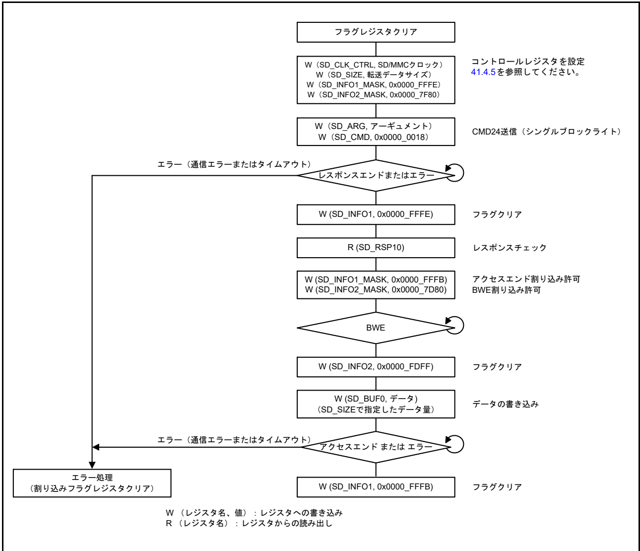
図 41.12 シングルブロックライト動作の例
