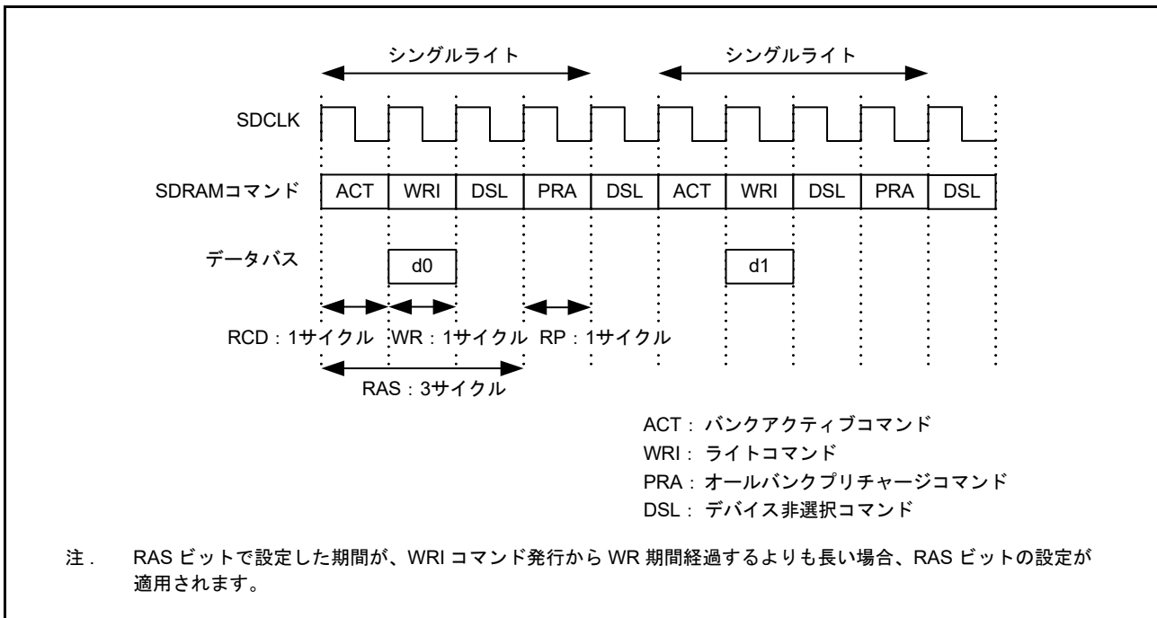
図 15.61 シングルライトタイミング例 (4)
