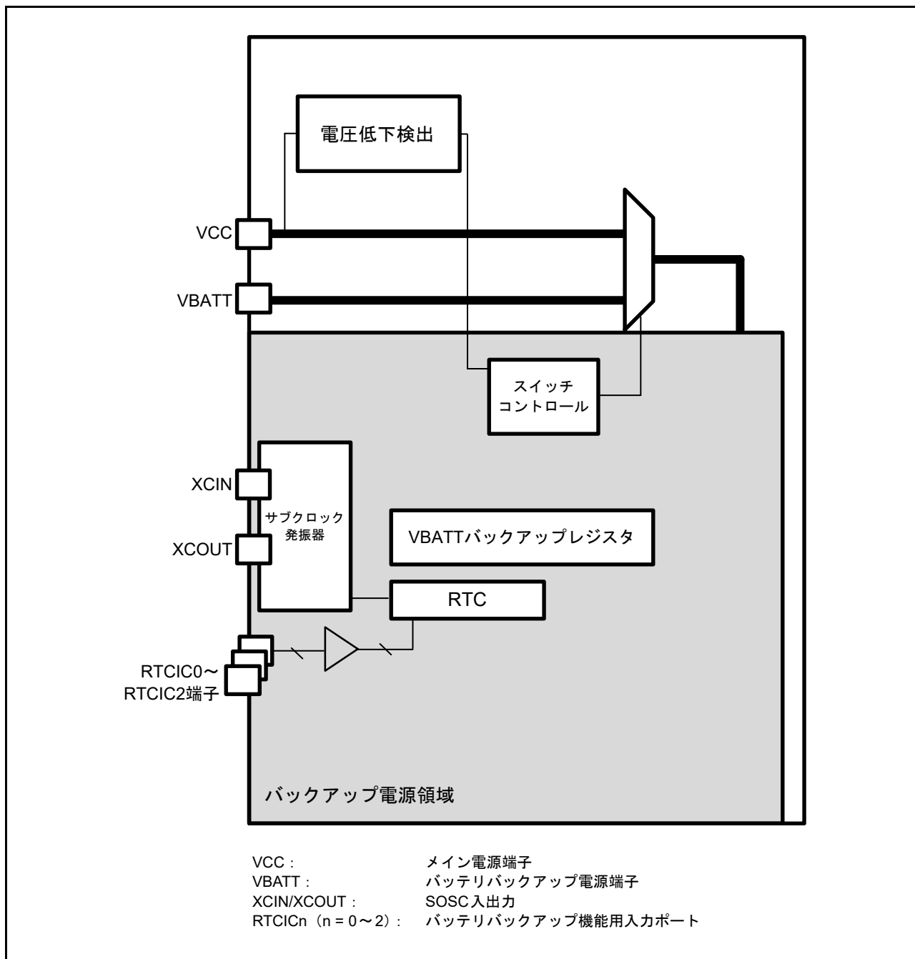
図 12.1 バッテリーバックアップ機能の構成図
