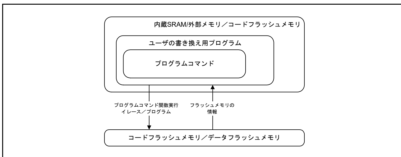
図 53.15 セルフプログラミングの概念
