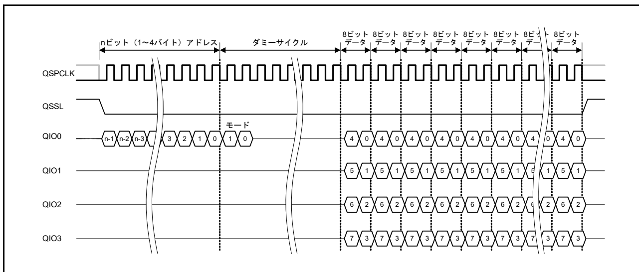
図 37.24 XIP モード時のファストリード Quad 出力バスサイクル
