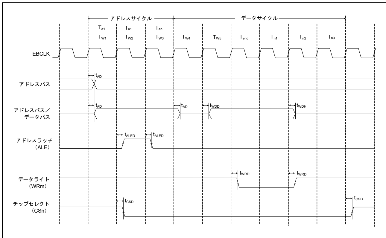
図 55.21 アドレス/データマルチプレクスバスのライトアクセスタイミング
