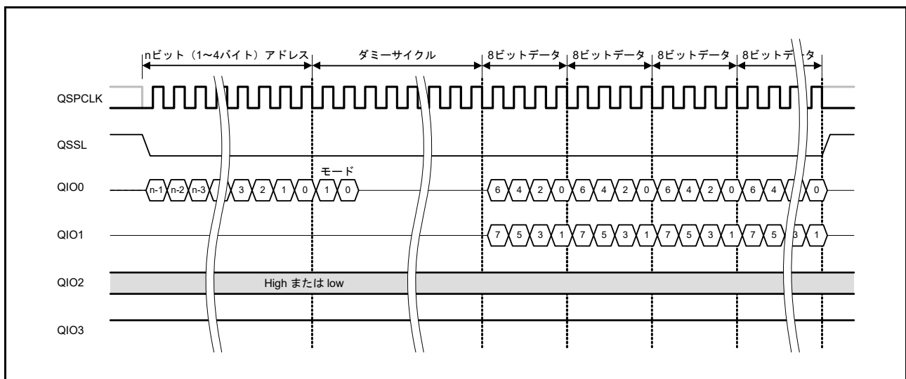
図 37.20 XIP モード時のファストリード Dual 出力バスサイクル
