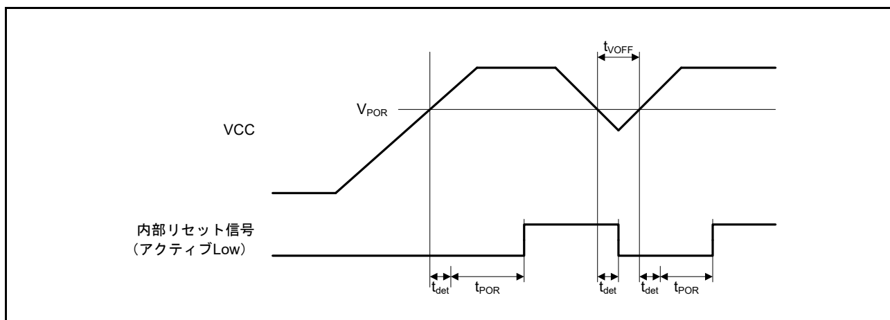
図 55.83 パワーオンリセットタイミング
