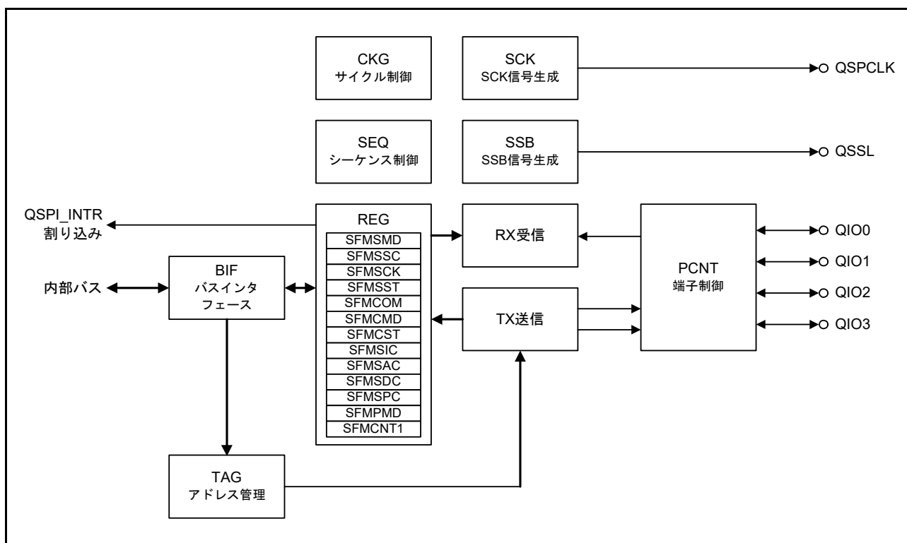
図 37.1 QSPIのブロック図
