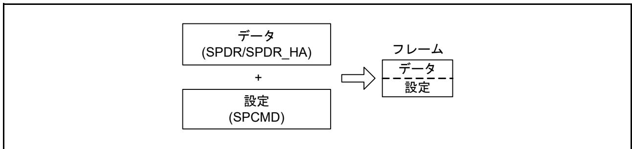
図 36.33 フレームの概念図
