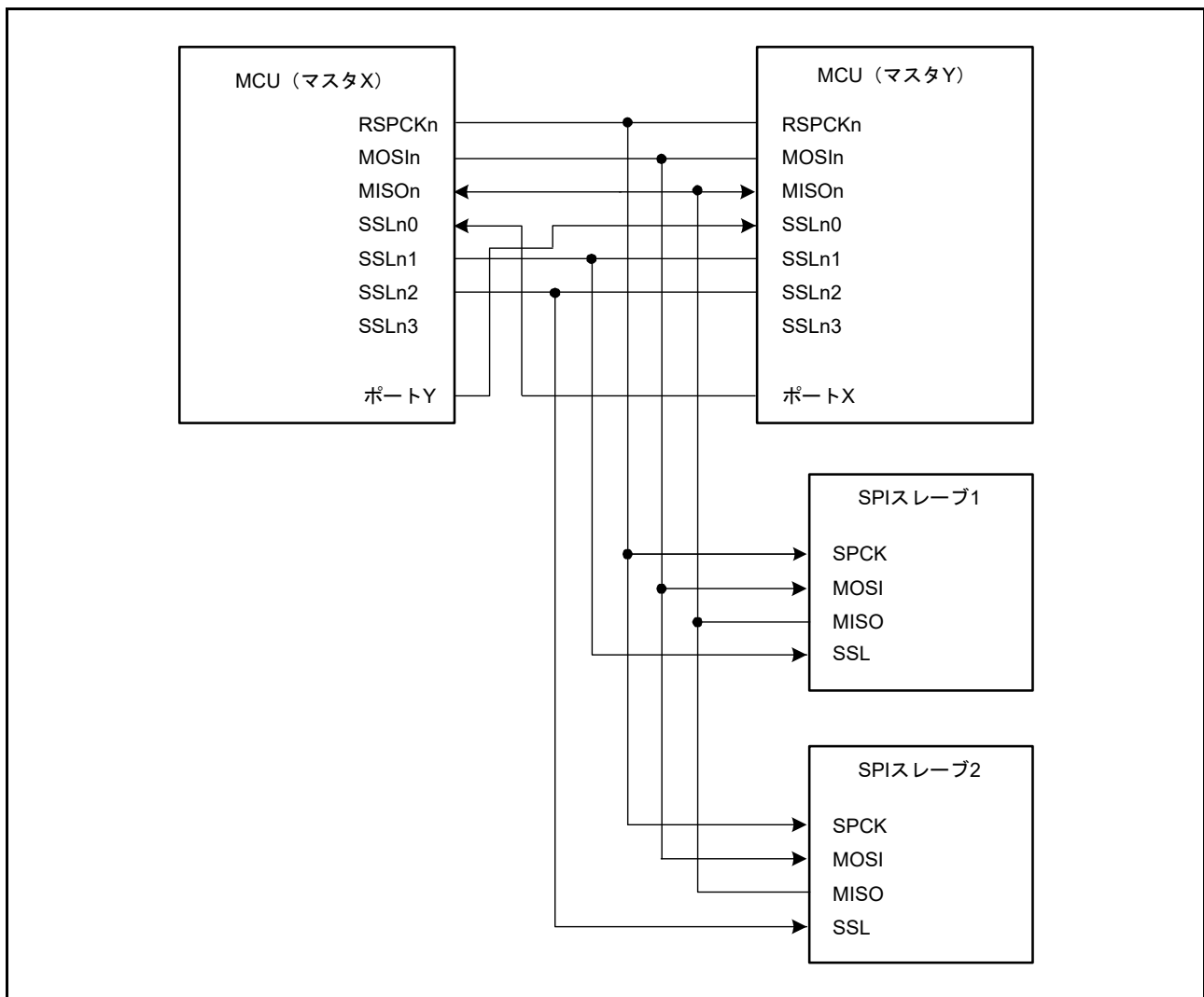
図 36.10 マルチマスタ/マルチスレーブの構成例 (MCU はマスタ)
