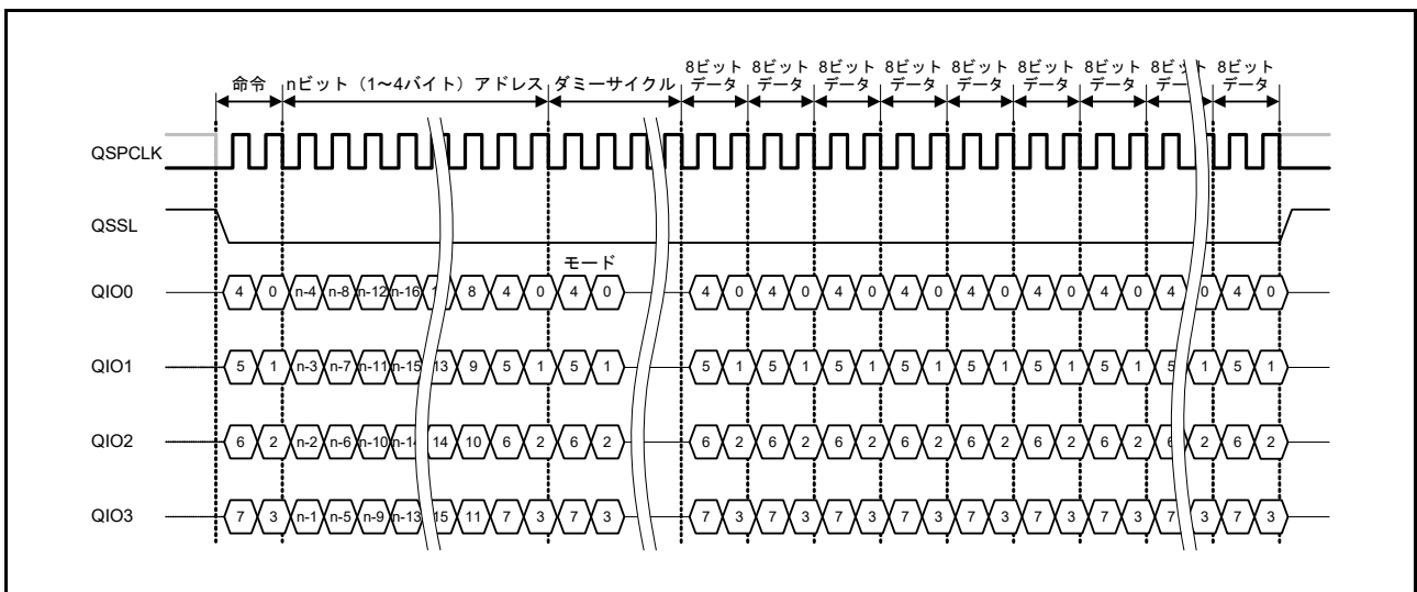
図 37.7 Quad-SPI プロトコル例 (ファストリード)
