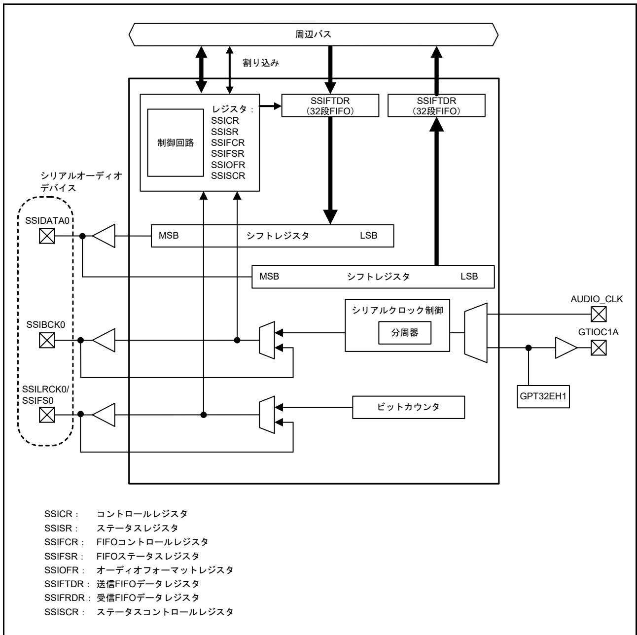
図 39.3 半二重通信の SSIE ブロック図 (SSIE0)
