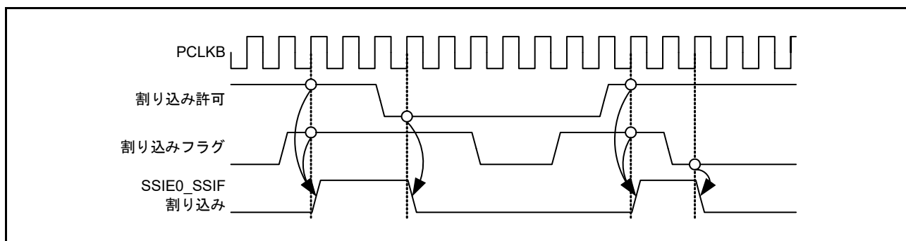
図 39.59 割り込み要因共通のタイミング図 (SSIE0_SSIF)
