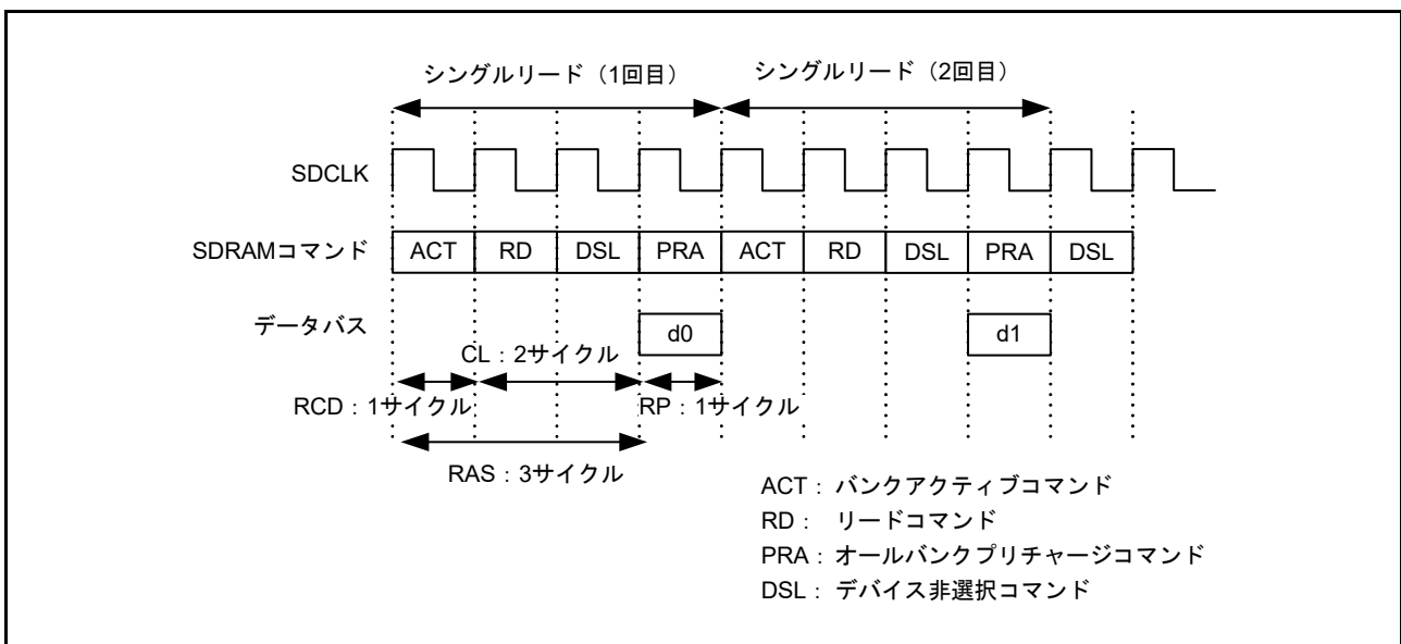
図 15.57 シングルリードタイミング例 (5) (1 転送要求に対して 2 回バスアクセスが発生する場合)
