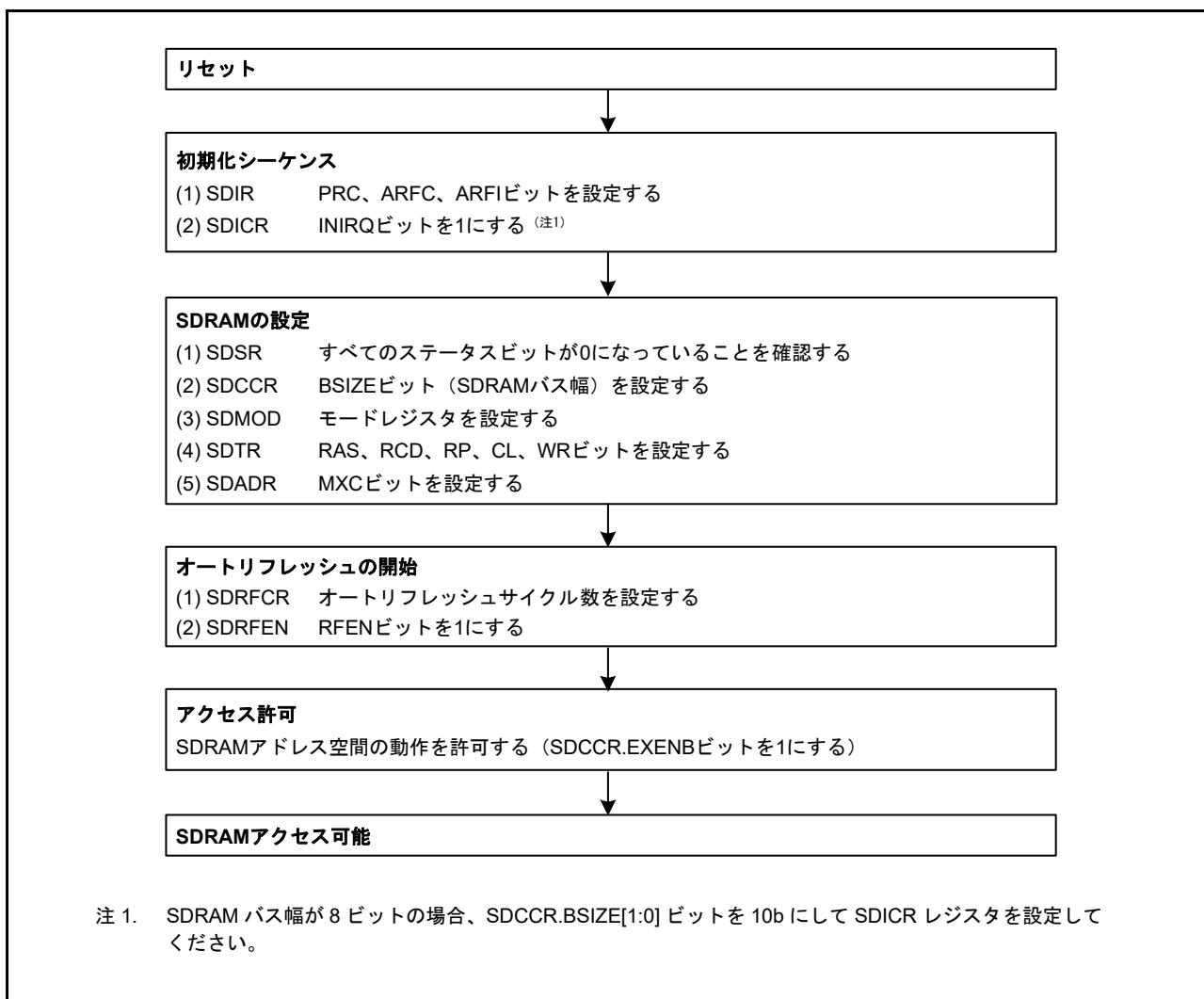
図 15.50 SDRAMC の設定手順
