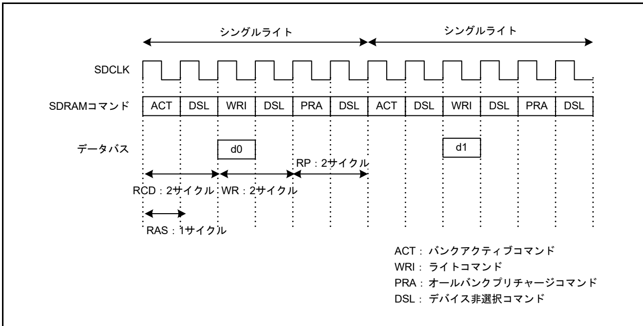
図 15.60 シングルライトタイミング例 (3)
