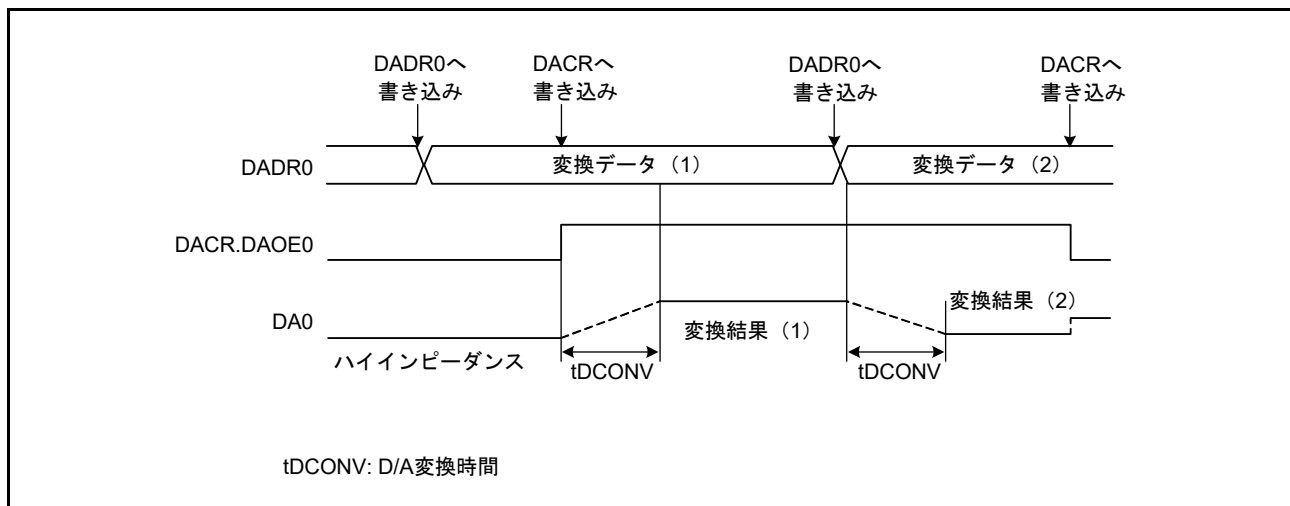
図 46.2 DAC12の動作例
