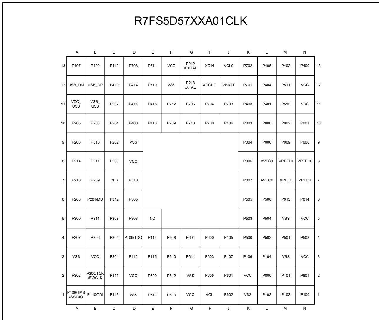
図 1.3 145-pin LGA のピン配置図 (上面図)
