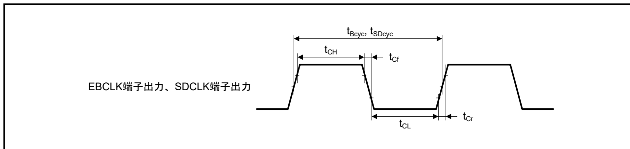
図 55.7 EBCLK および SDCLK の出力タイミング
