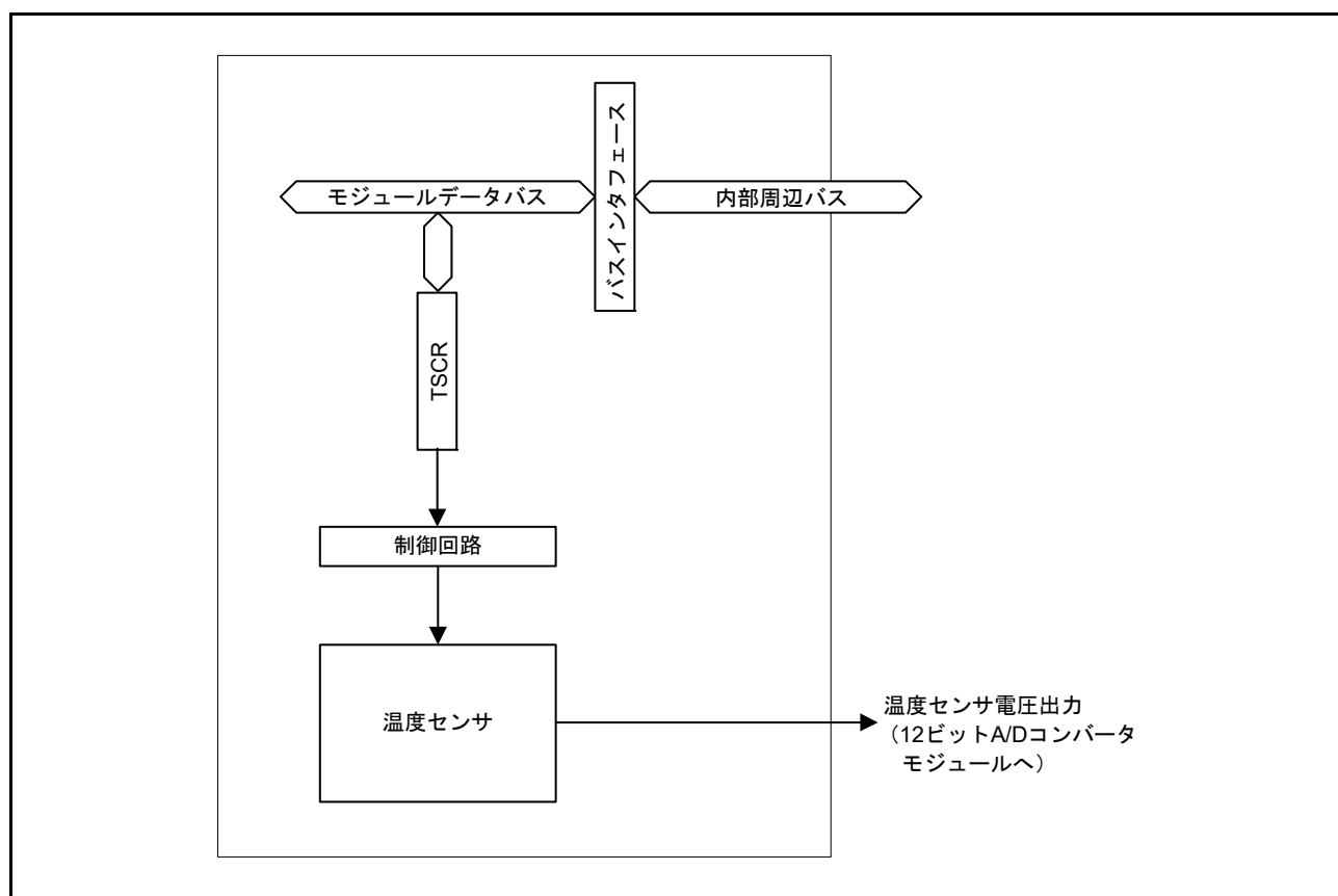
図 47.1 温度センサのブロック図
