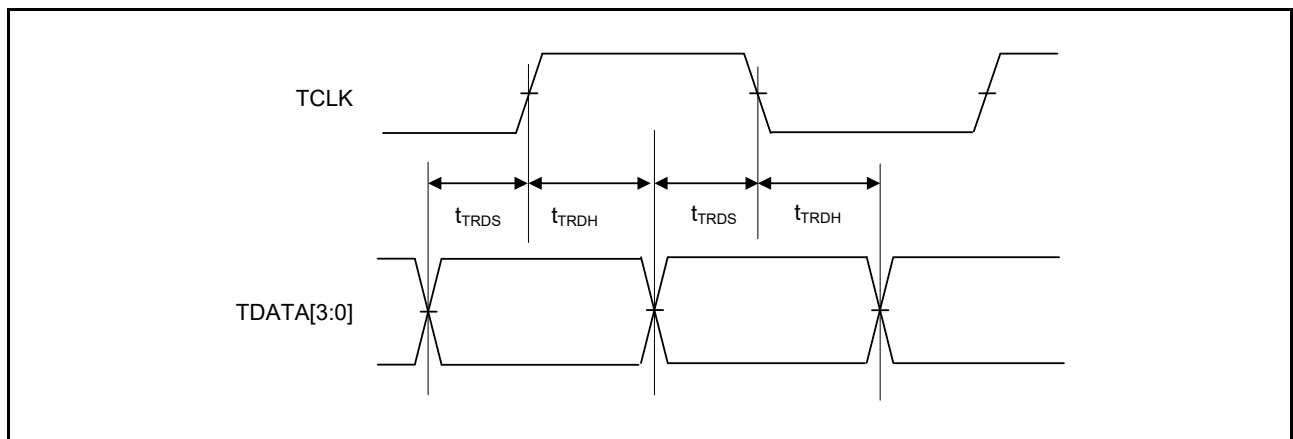
図 55.97 ETM 出力タイミング
