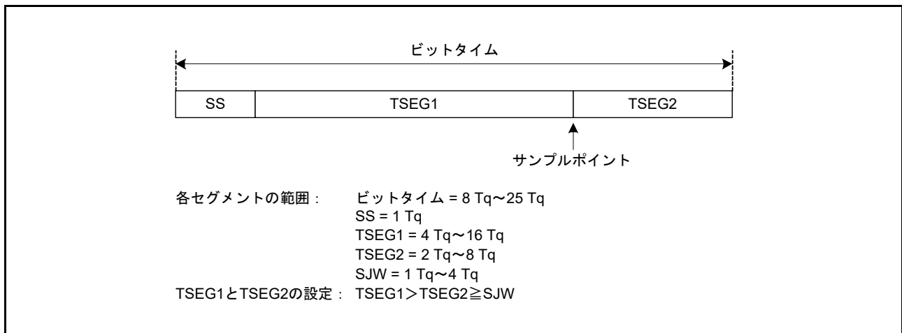
図 35.12 ビットタイミング
