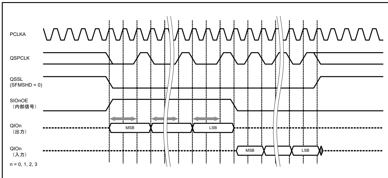
図 37.13 SFMOSW ビットを使用したシリアルデータ出力のセットアップ時間調整
