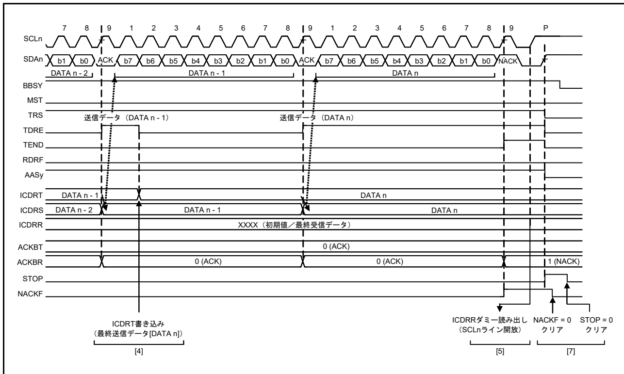
図 34.17 スレーブ送信の動作タイミング (2)
