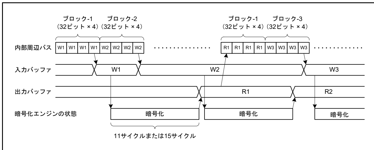
図 44.3 暗号化と復号タイミング (AES)
