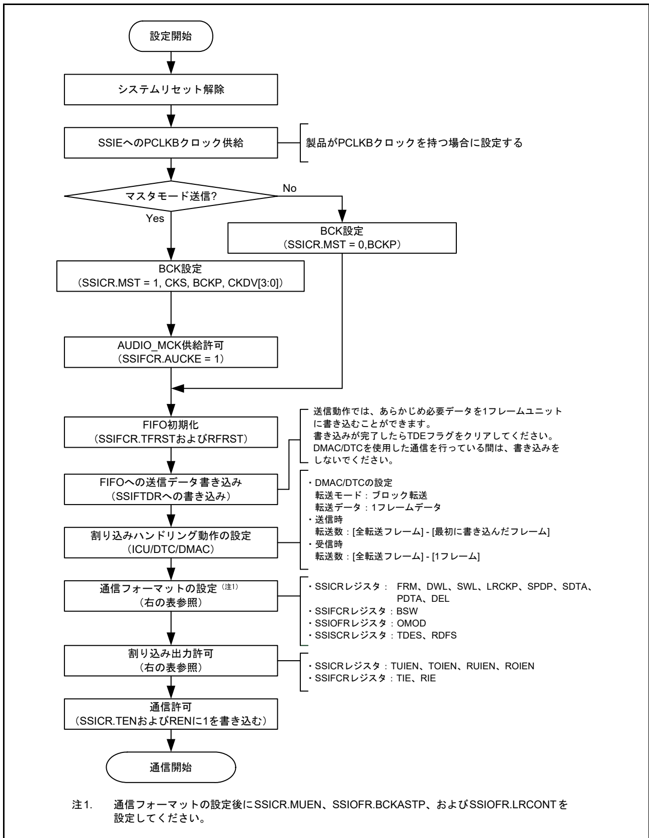
図 39.53 通信開始手順 (CPU 動作手順)
