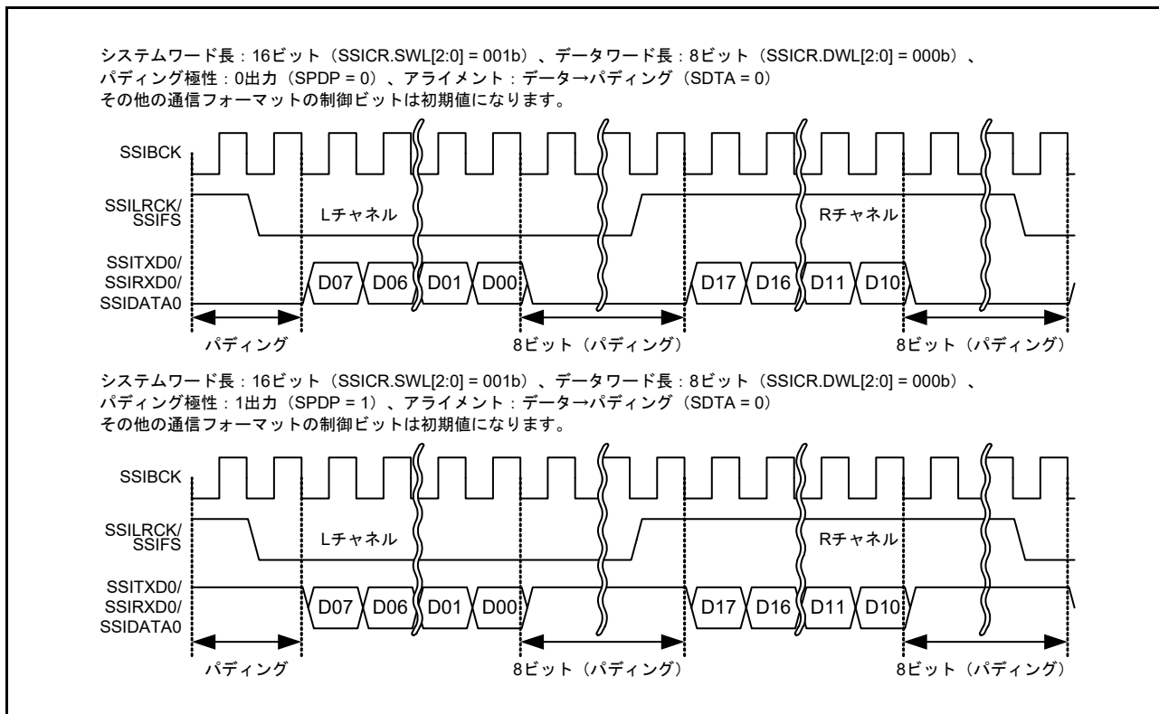
図 39.11 パディングビット極性
