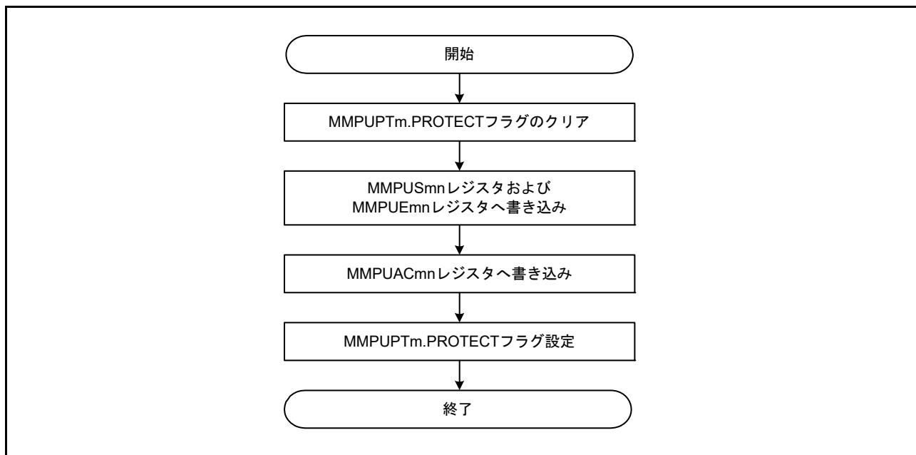
図 16.8 領域追加のレジスタ設定フロー
