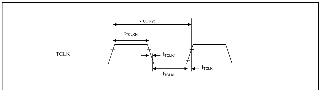
図 55.96 ETM TCLK タイミング
