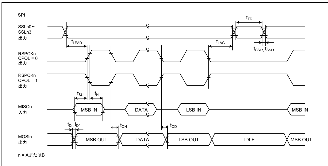
図 55.49 CPHA = 0 の場合におけるマスタの SPI タイミング
