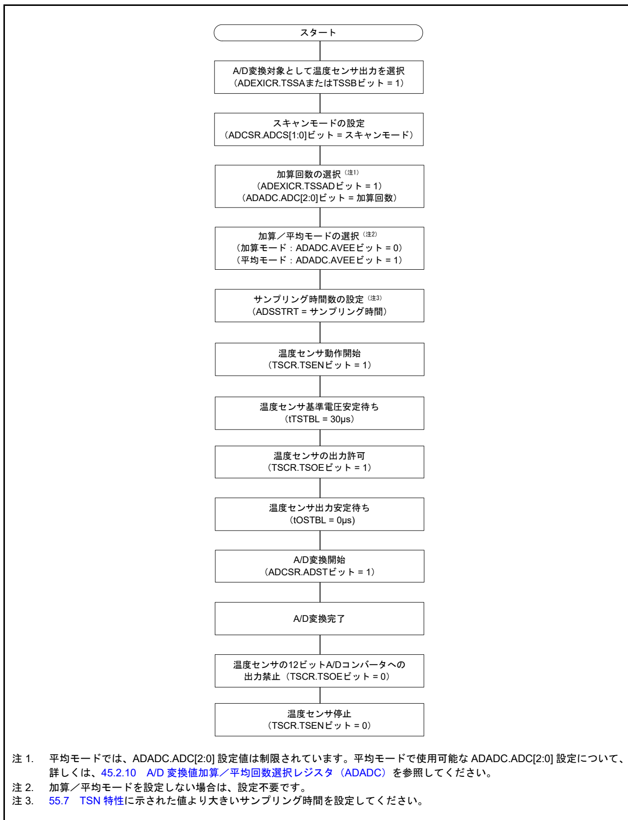
図 47.2 温度センサの使用手順
