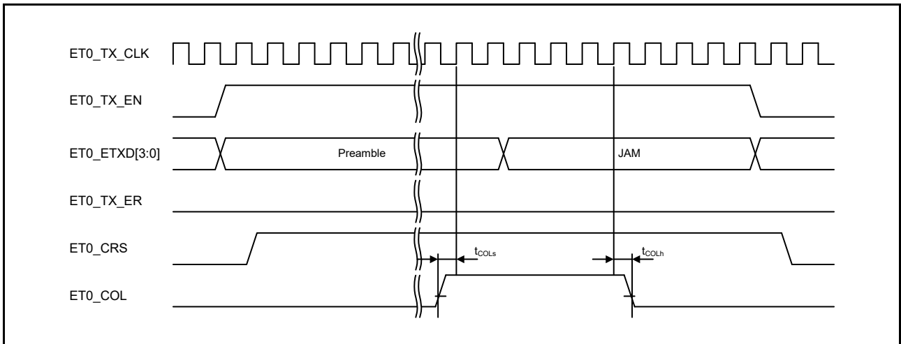
図 55.70 競合発生時の MII 送信タイミング
