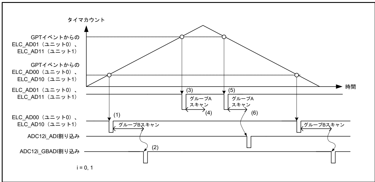
図 45.24 グループスキャンモードでダブルトリガモードを使用する場合の基本動作例 (ELC からの同期トリガ使用時)
