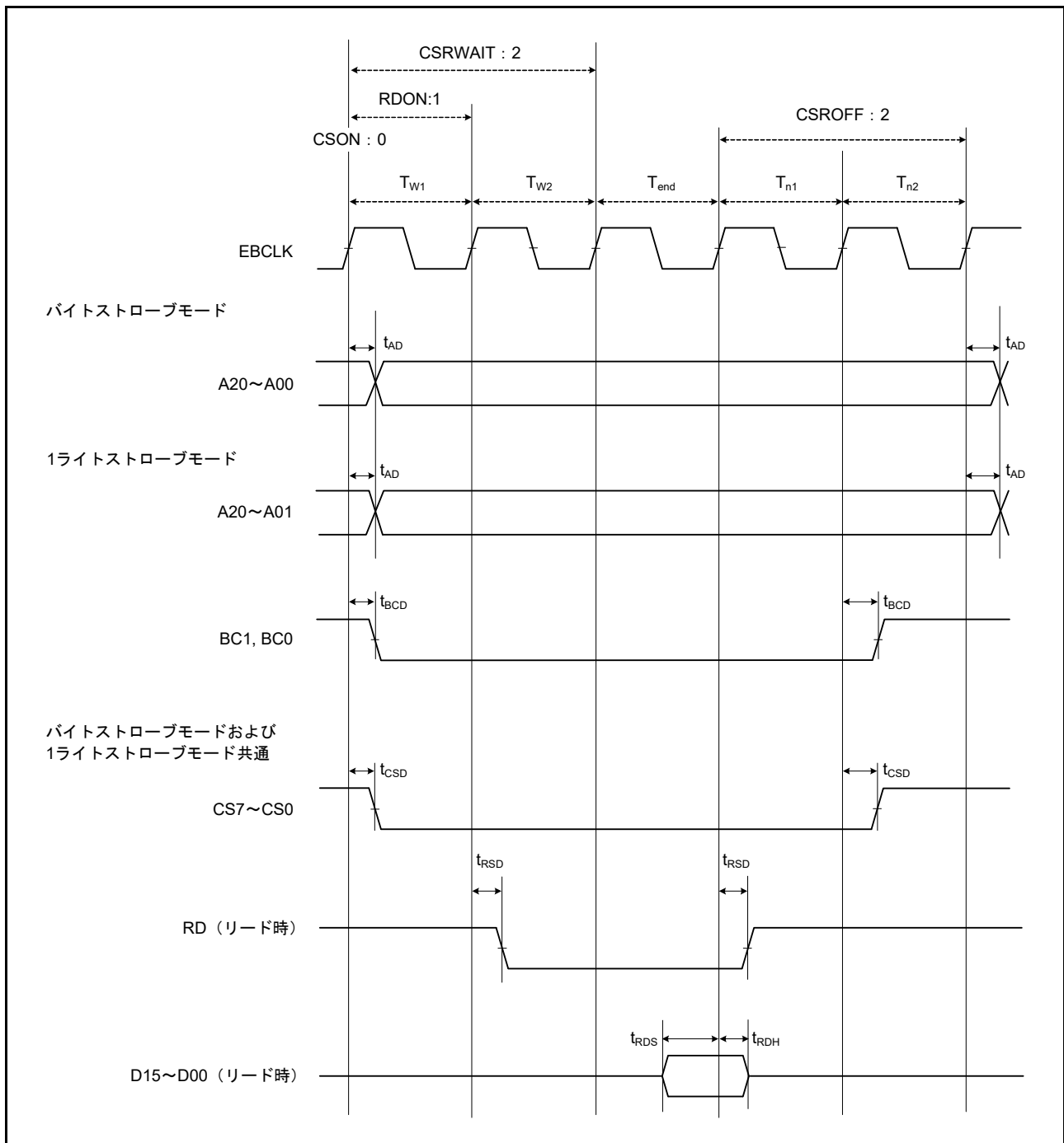
図 55.22 バスクロック同期を使用したノーマルリードサイクルの外部バスタイミング
