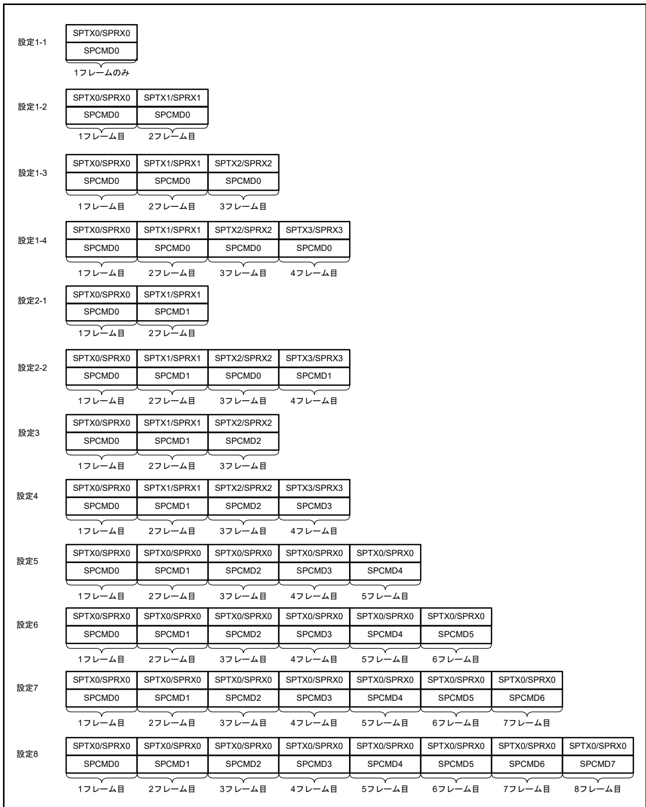
図 36.34 シーケンス動作時の SPI コマンドレジスタと送受信バッファの対応関係
