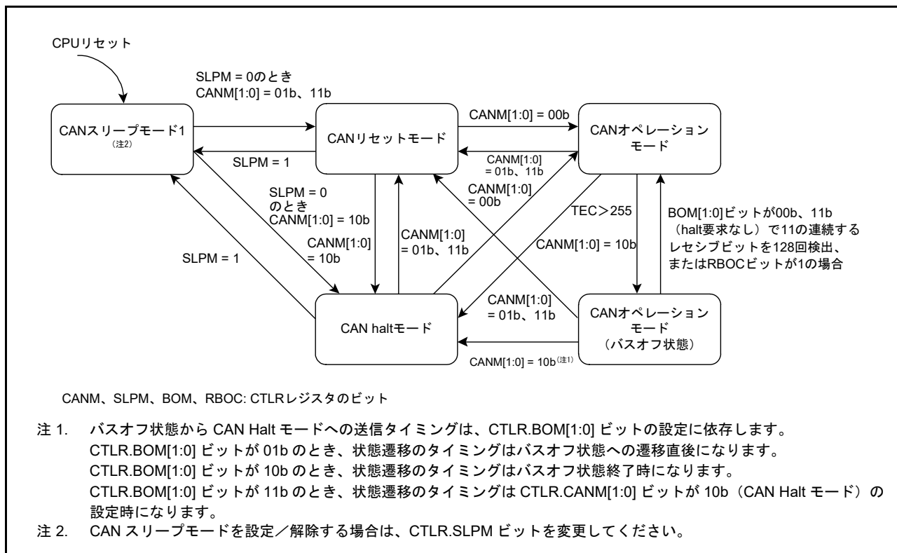
図 35.9 各動作モード間の遷移
