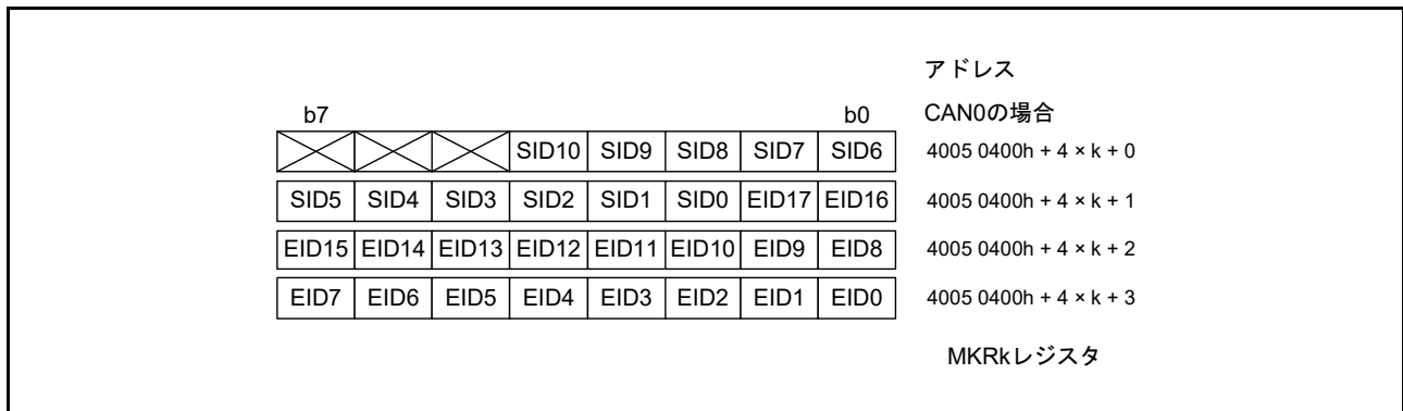
図 35.14 MKRk レジスタの構成 (k = 0 ~ 7)
