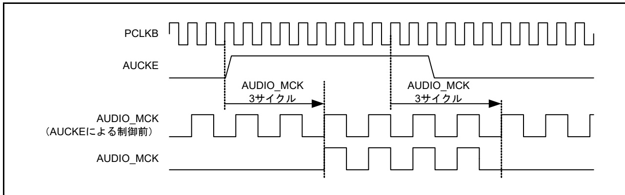
図 39.25 AUDIO_MCK の停止/再開
