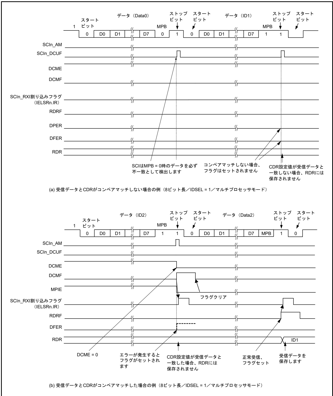
図 32.6 アドレス一致検出の例 (2) (マルチプロセッサモード)
