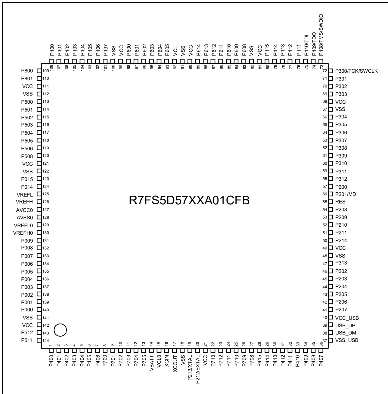
図 1.4 144-pin LQFP のピン配置図 (上面図)
