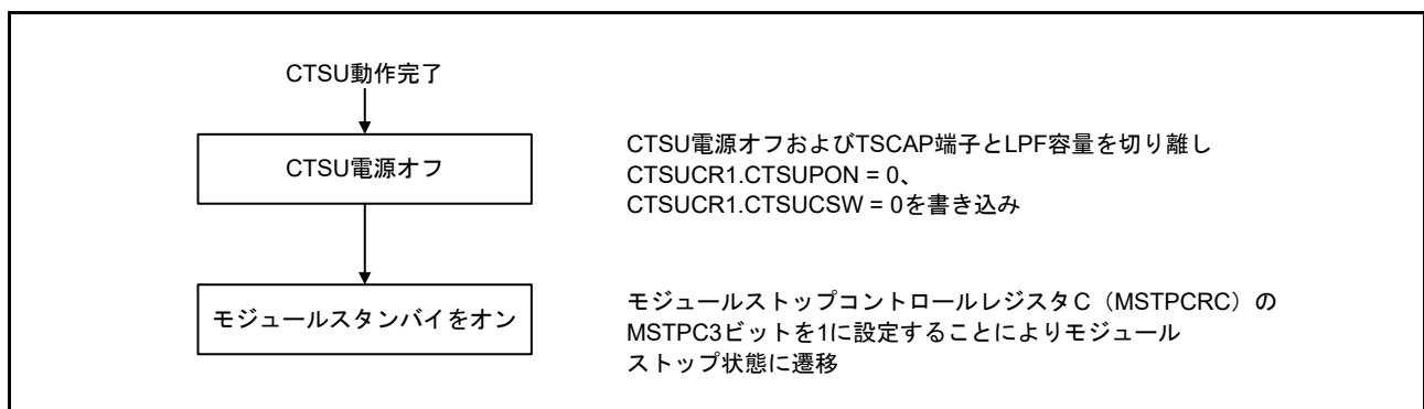
図 49.10 CTSUS 停止フロー
