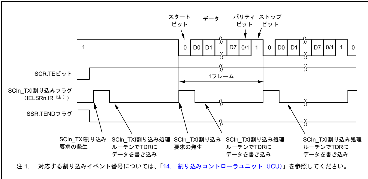
図 32.9 調歩同期式モードにおけるシリアル送信の動作例 (1) (8 ビットデータ/パリティあり/1ストップビット/CTS 機能不使用/送信開始時)
