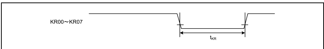
図 55.39 キー割り込み入力タイミング
