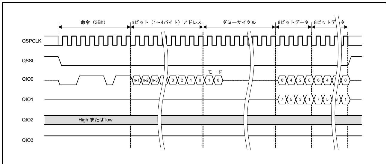
図 37.19 ファストリード Dual 出力バスサイクル
