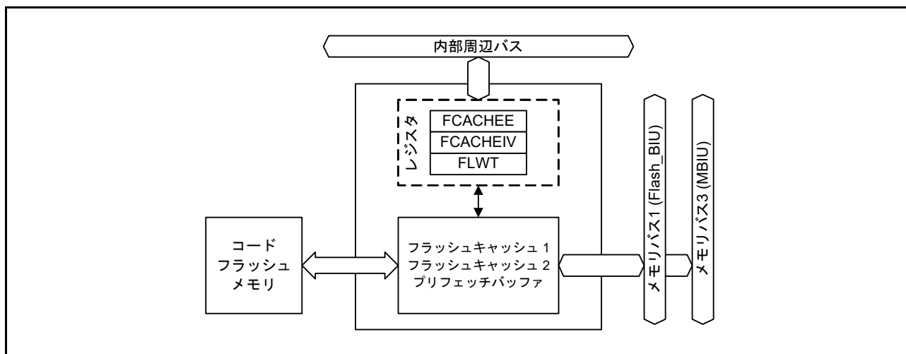
図 53.4 FCACHE のブロック図
