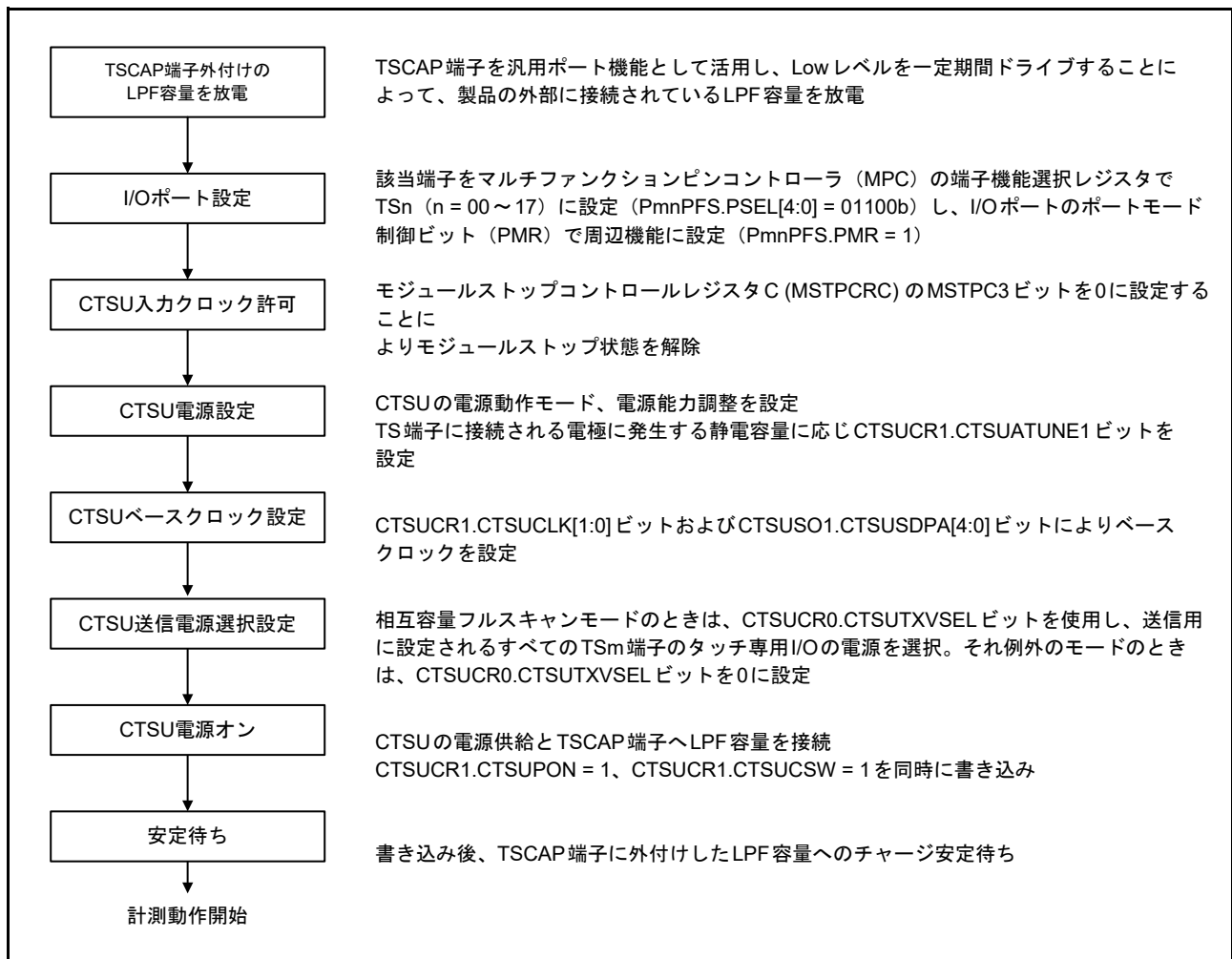
図 49.9 CTSUS 初期設定フロー
