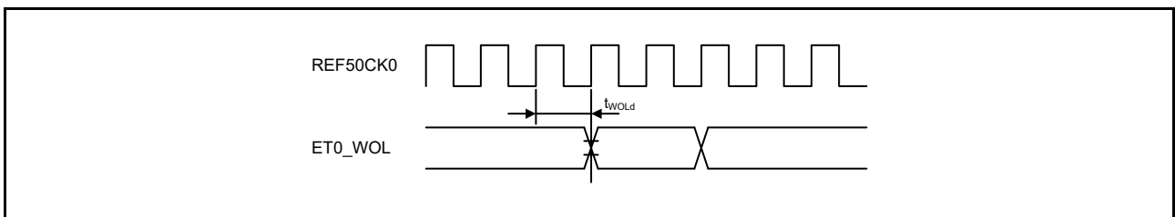
図 55.68 RMI に対する WOL 出力タイミング
