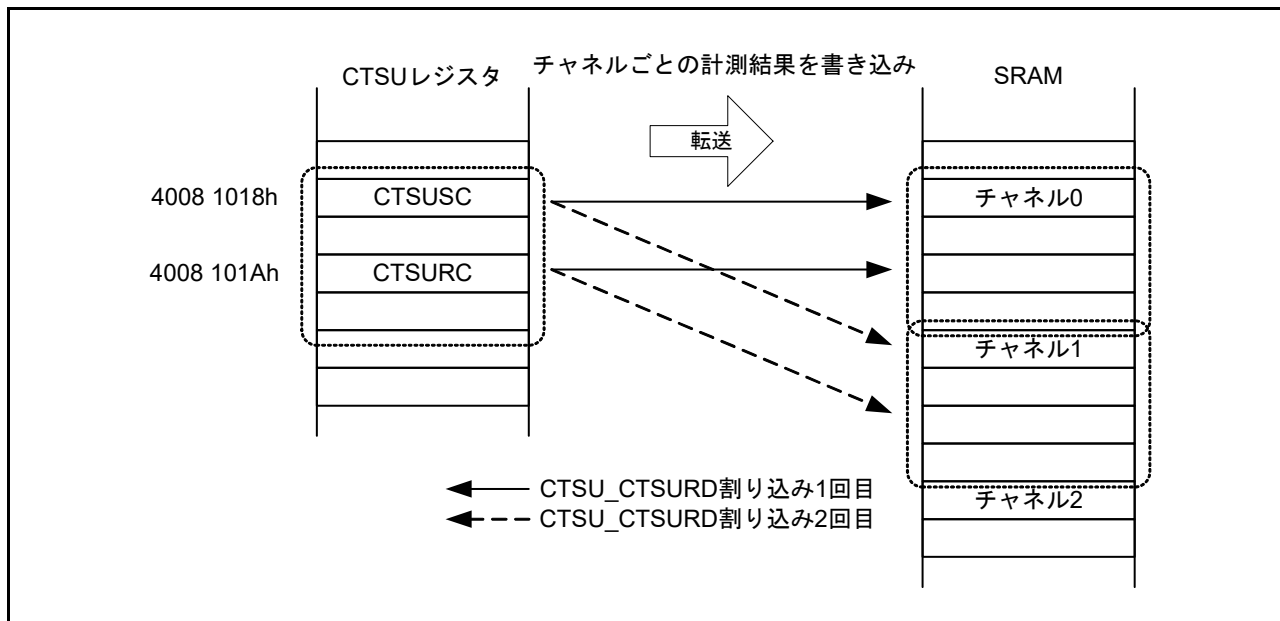
図 49.20 CTSU_CTSURD 割り込みを用いた DTC 転送動作例
