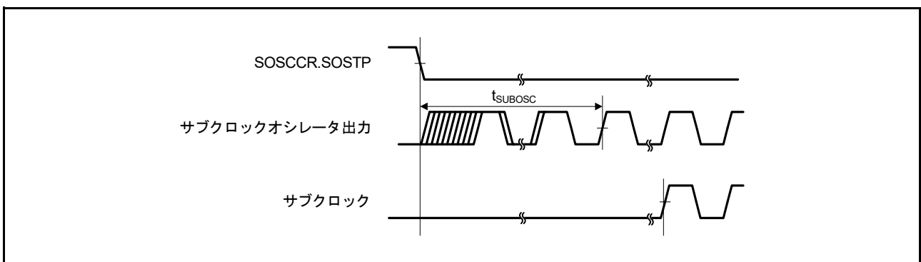
図 55.12 サブクロック発振開始タイミング
