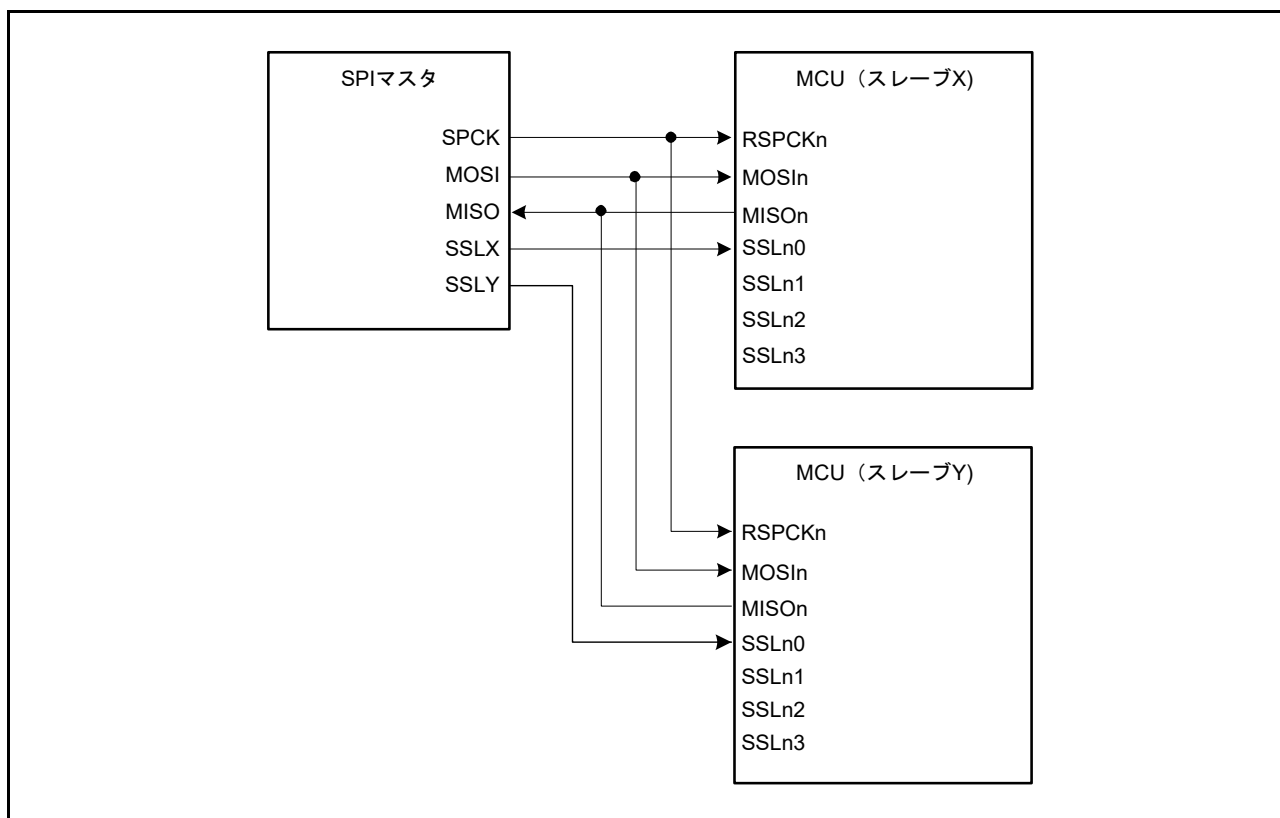
図 36.9 シングルマスタ/マルチスレーブの構成例 (MCU はスレーブ)
