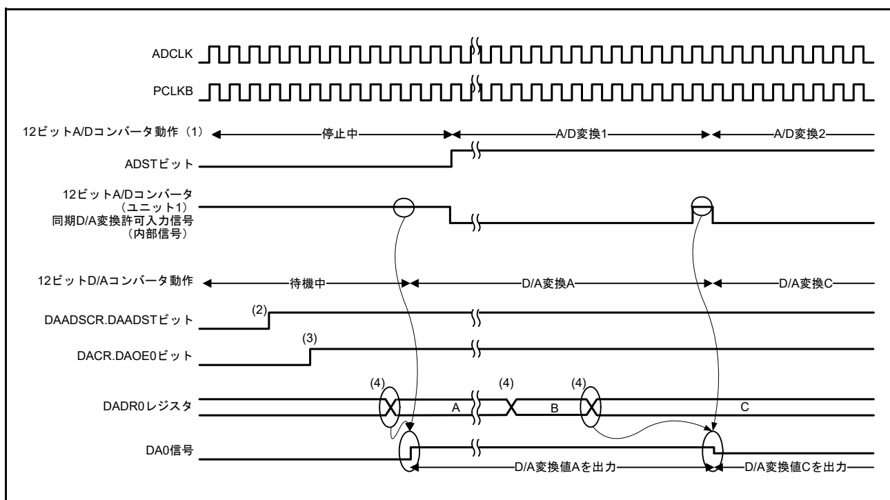
図 46.3 DAC12 を ADC12 に同期して変換する例
