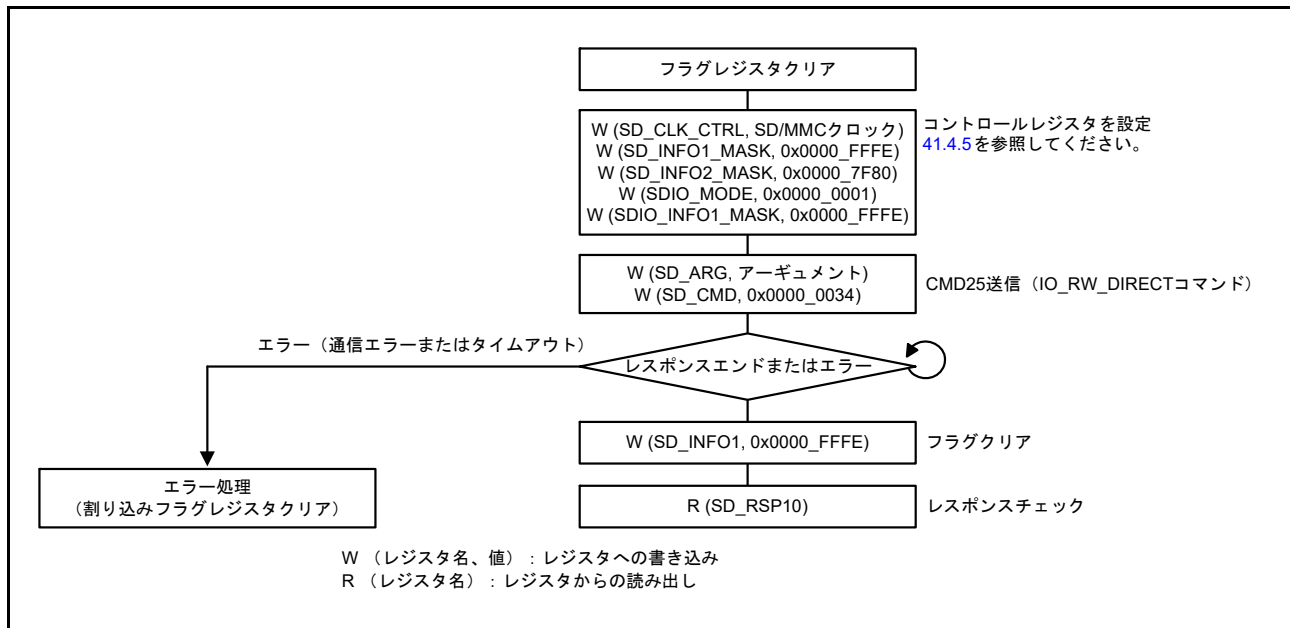
図 41.16 IO_RW_DIRECT コマンド (CMD52) 動作の例
