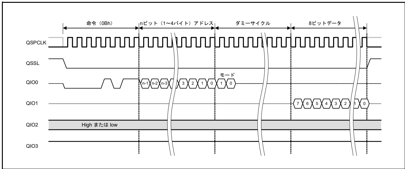
図 37.17 ファストリードバスサイクル
