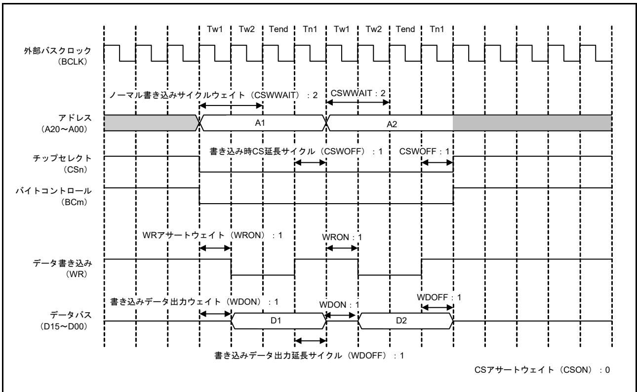
図 15.15 ノーマルライトアクセスの動作例 (1 転送要求に対して 2 回バスアクセスが発生する場合 : 1 ライトストロープモード時) (n = 0 ~ 7 および m = 0, 1)
