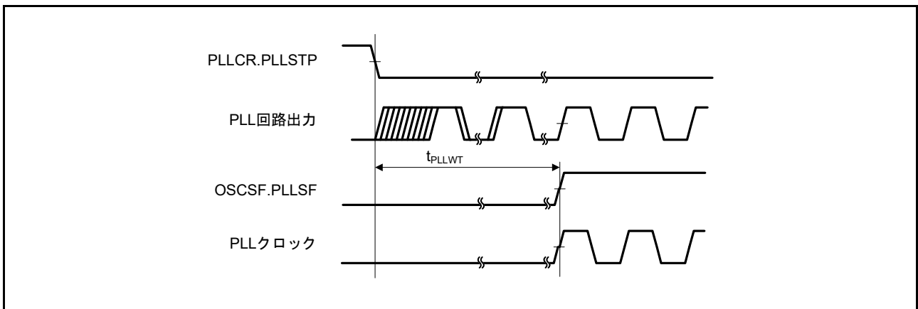
図 55.11 PLL クロック発振開始タイミング
