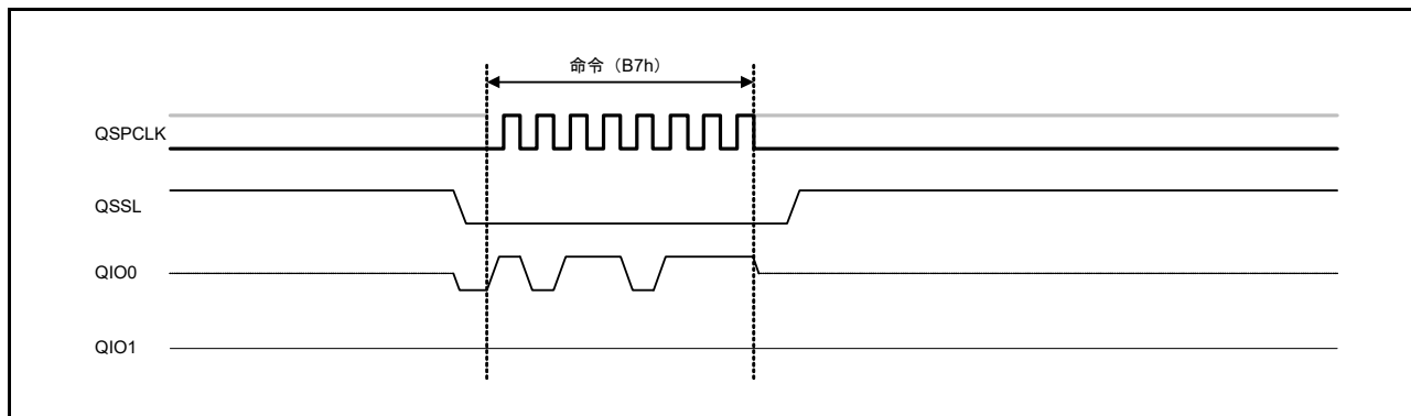
図 37.27 4 バイトモード遷移バスサイクル
