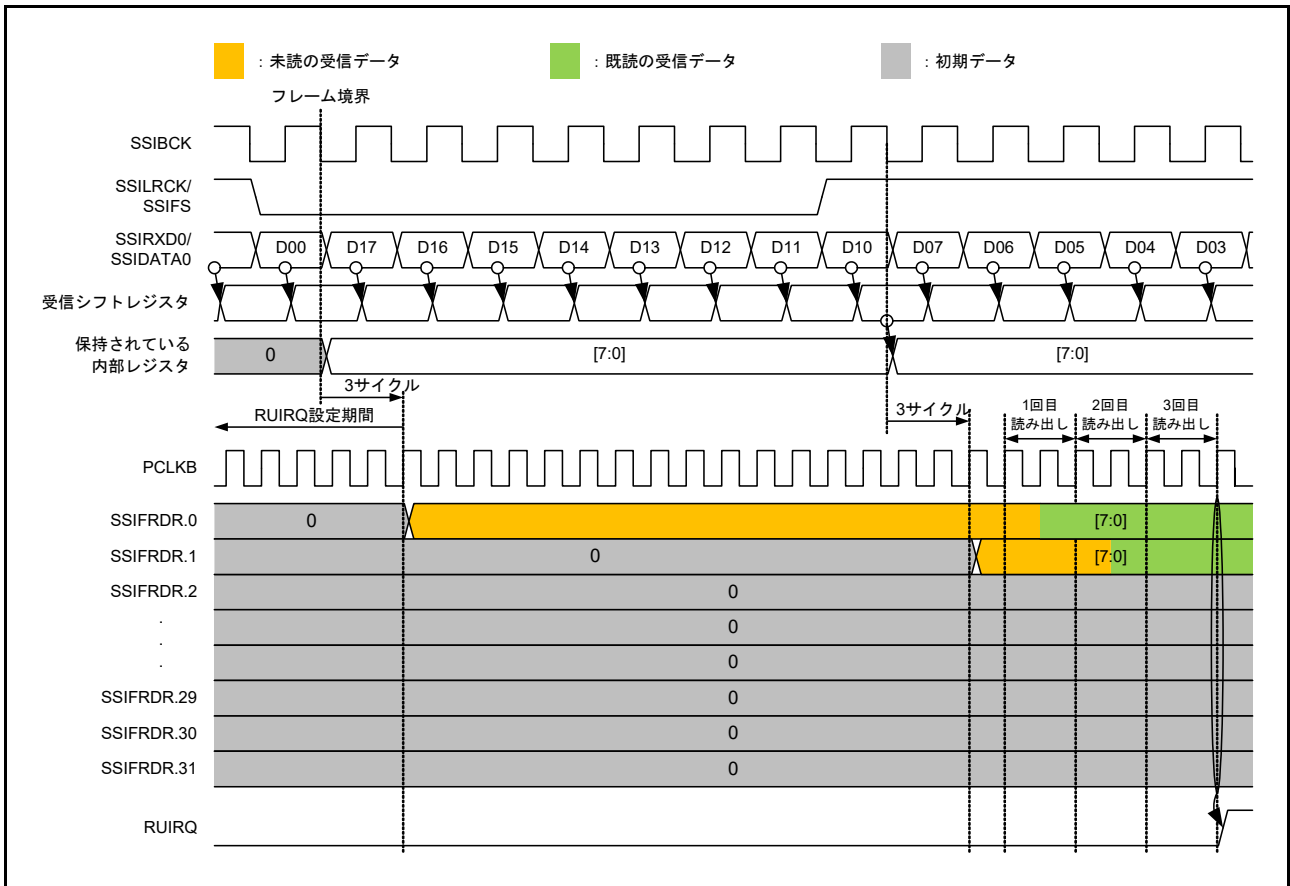
図 39.17 RUIRQ 設定タイミング
