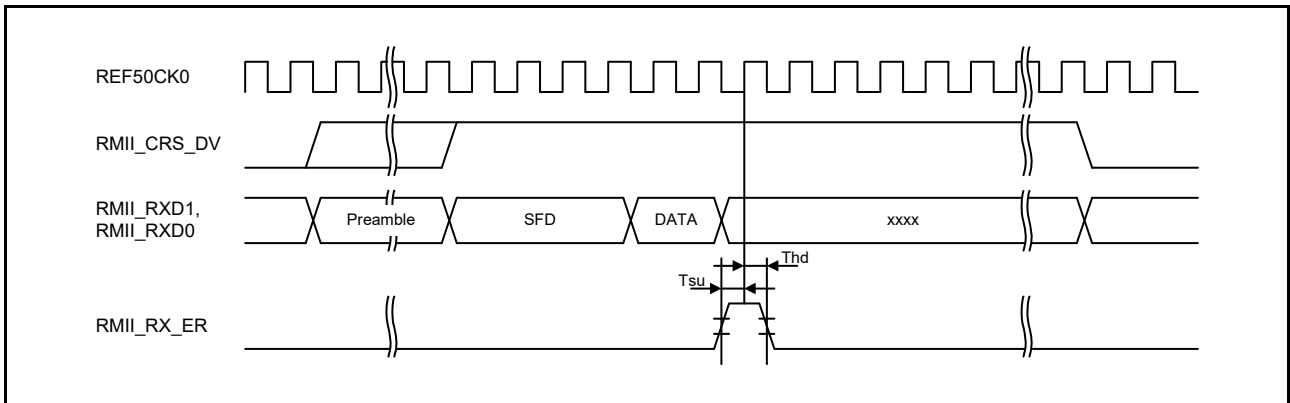
図 55.67 エラー発生時の RMI 受信タイミング
