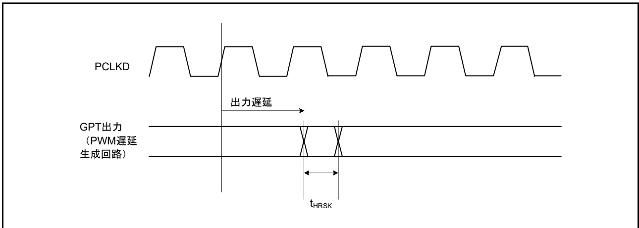
図 55.36 GPT (PWM 遅延生成回路) 出力遅延スキュー
