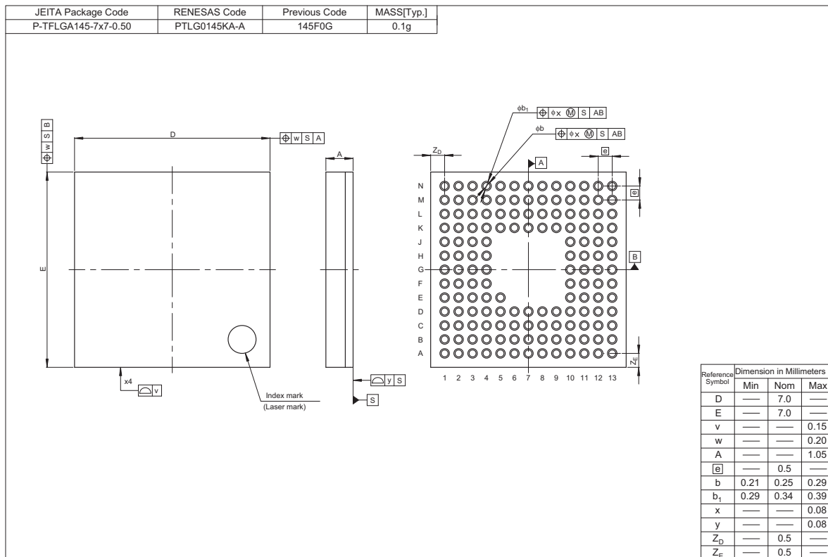
図 2.1 145 ピン LGA
