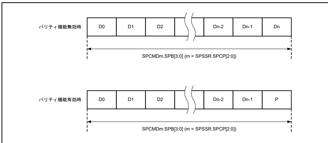
図 36.13 パリティ機能無効時と有効時のデータフォーマット
