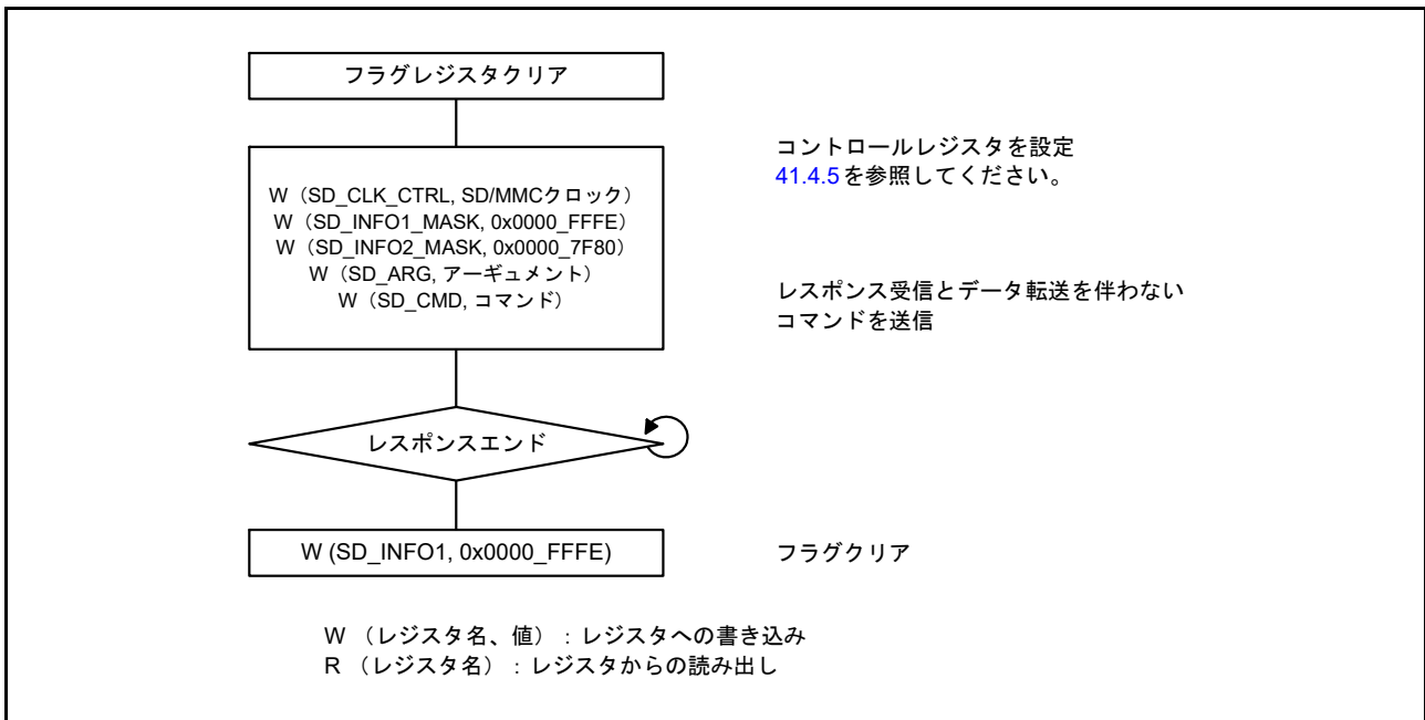
図 41.9 レスポンスまたはデータがないコマンドのフロー例
