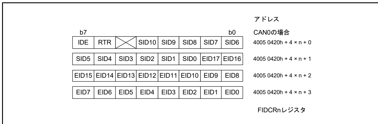
図 35.15 FIDCRn レジスタの構成 (n = 0, 1)
