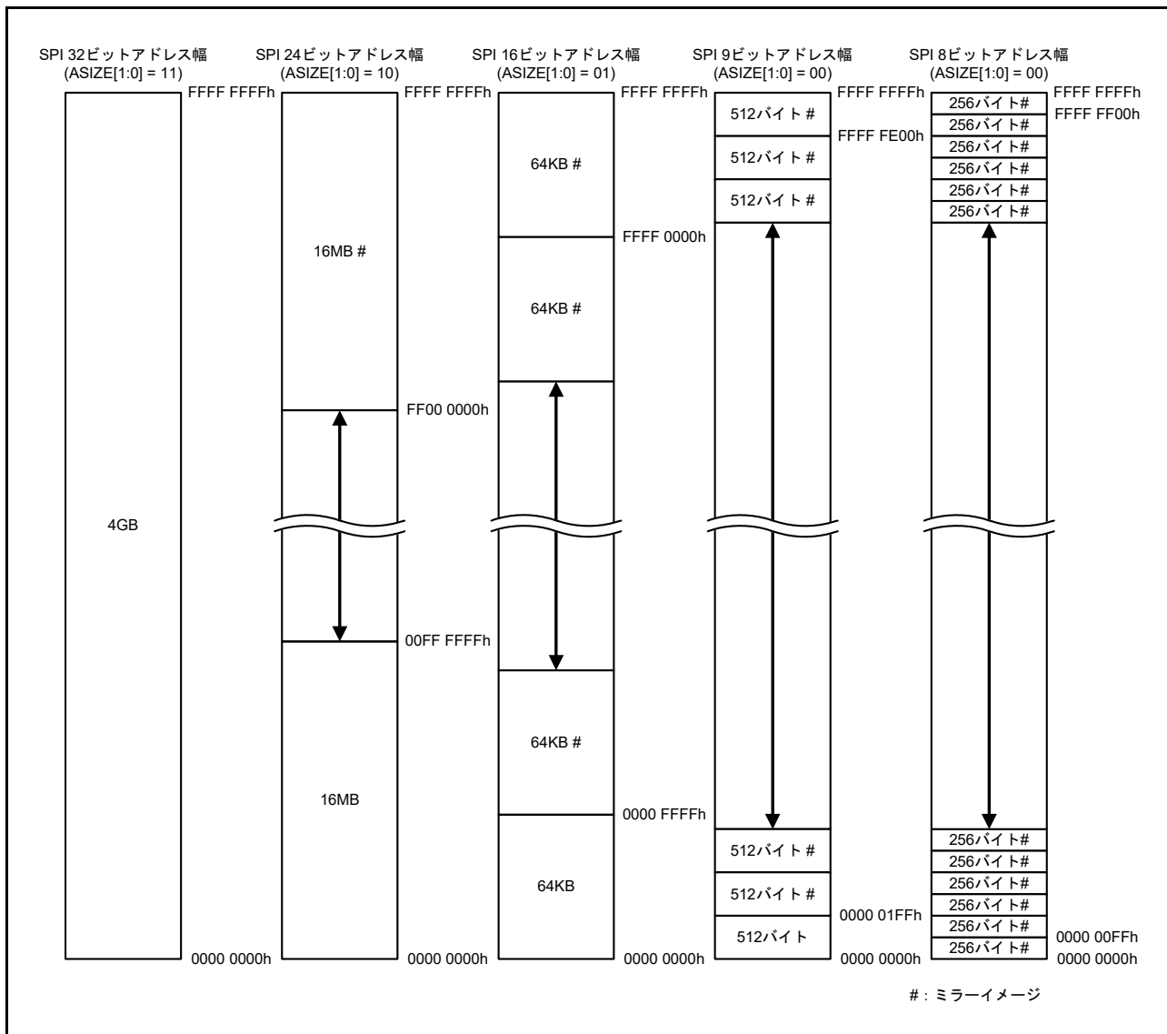
図 37.3 SPI 空間のメモリマップ
