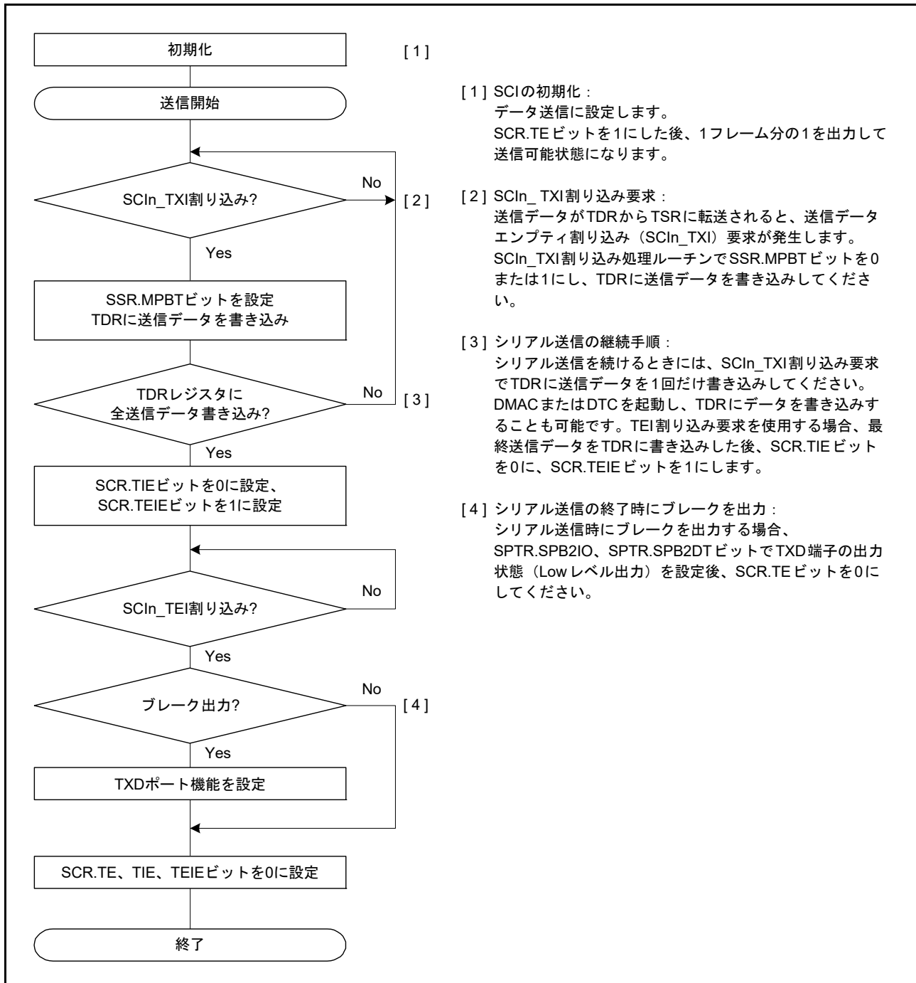
図 32.23 マルチプロセッサシリアル送信のフローチャート例 (非 FIFO 選択時)
