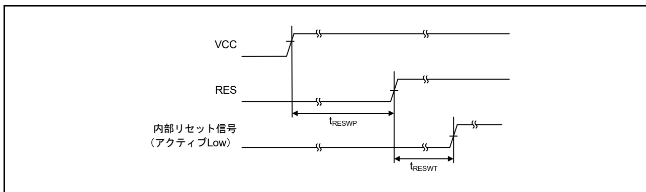
図 55.13 パワーオンリセットタイミング
