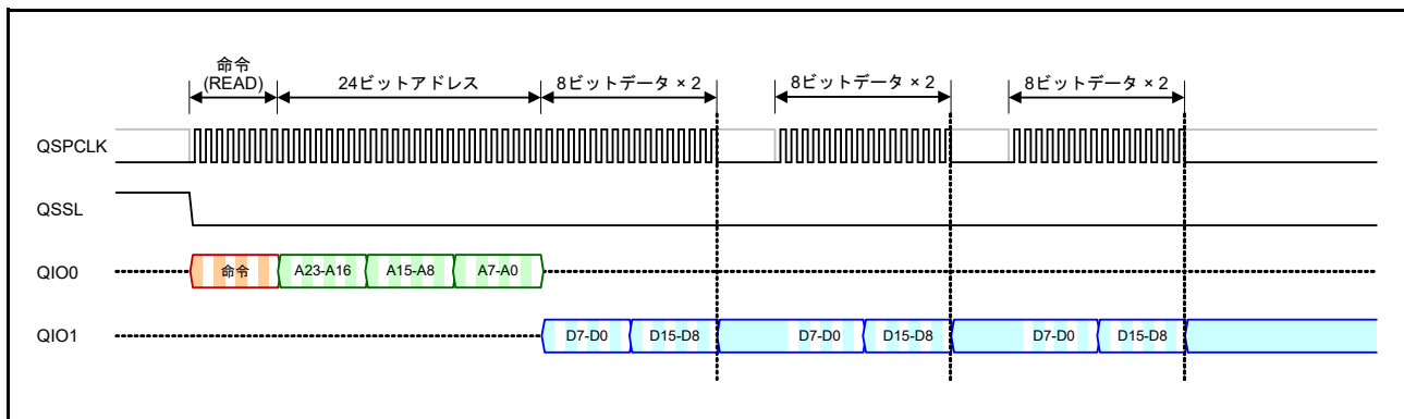
図 37.32 SPI バスサイクル拡張を使用した連続データのリード動作
