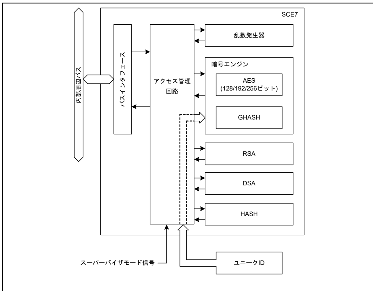
図 44.1 SCE7 ブロック図
