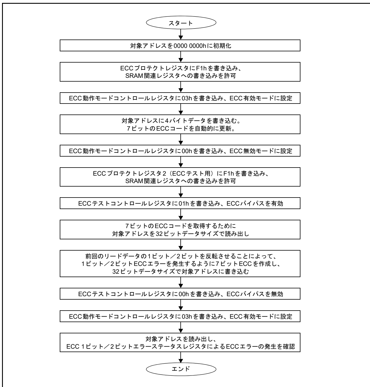
図 51.1 ECC デコーダのテスト方法
