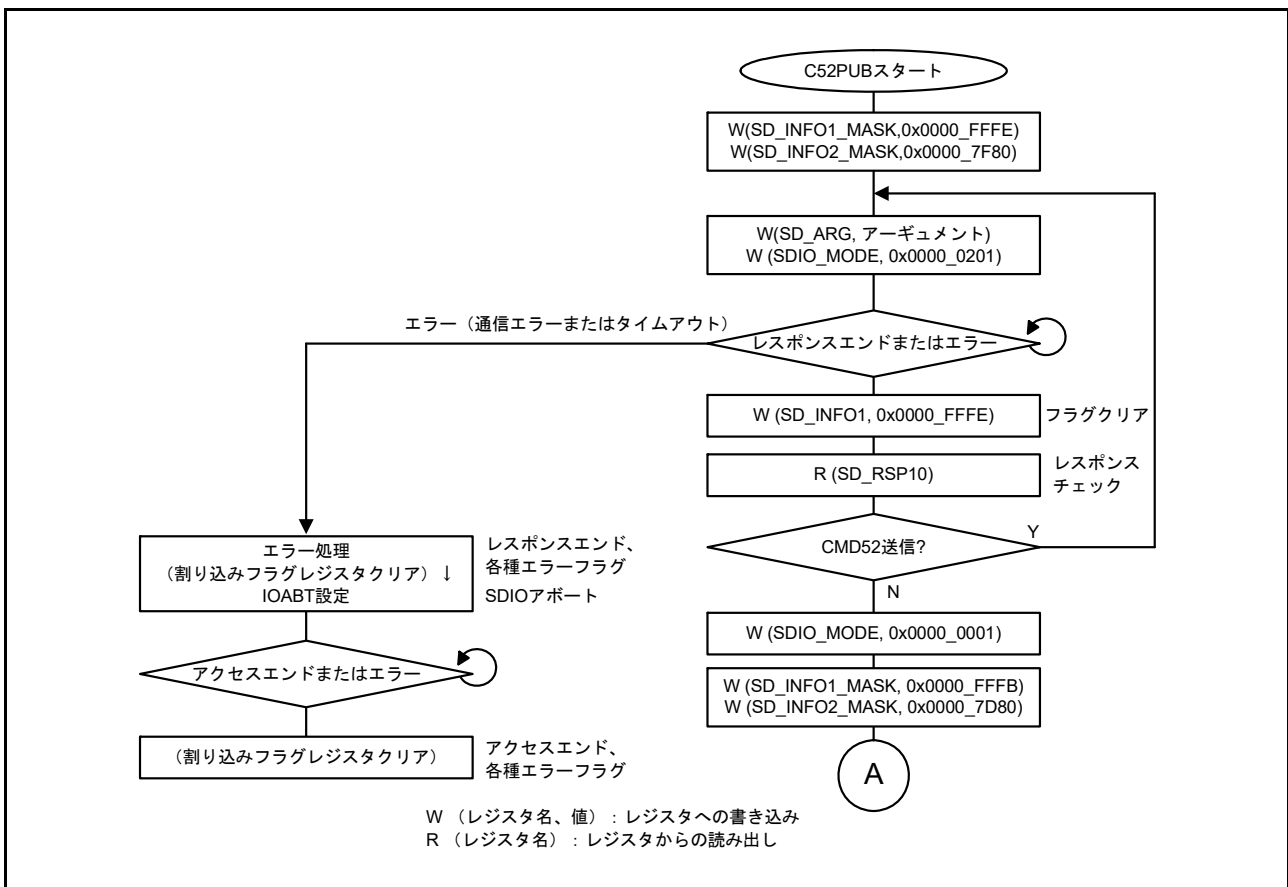
図 41.22 CMD53 マルチブロックライト時に CMD52 (SDIO none abort) が送信される場合のフロー
