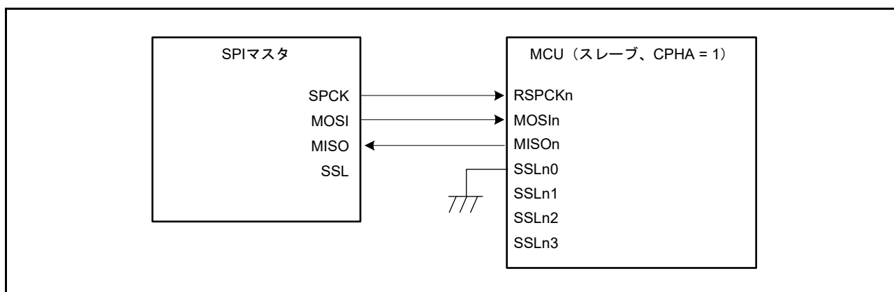
図 36.7 シングルマスタ/シングルスレーブの構成例 (MCU はスレーブ、CPHA = 1)
