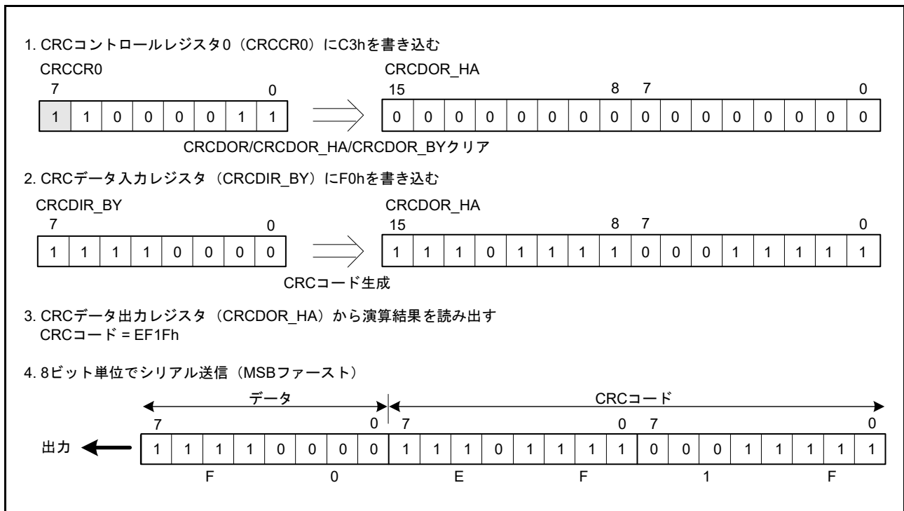
図 38.3 MSB ファーストのデータ送信
