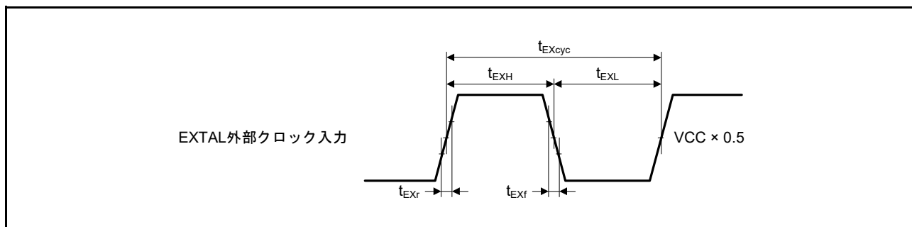
図 55.8 EXTAL 外部クロック入力タイミング
