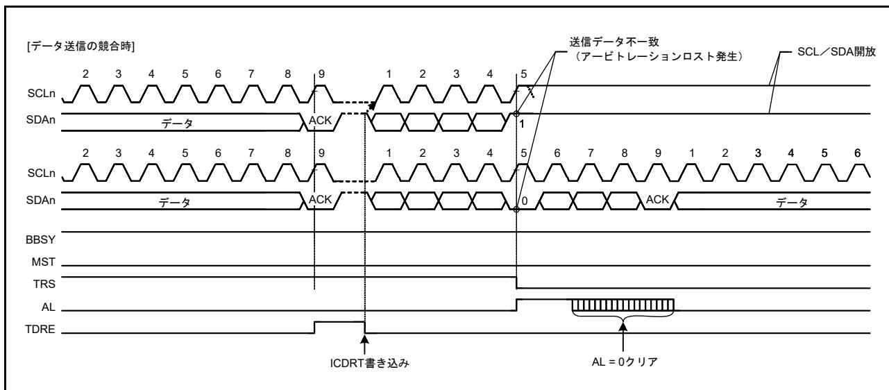
図 34.44 スレーブアービトレーションロスト検出の動作例 (SALE = 1 の場合)
