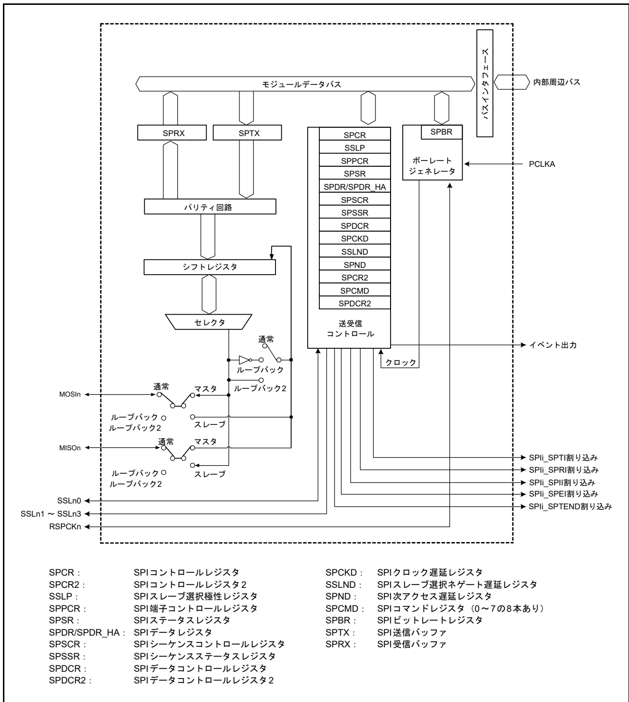
図 36.1 SPIのブロック図
