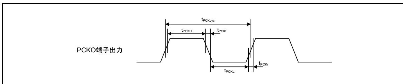
図 55.75 PDC 出力クロックタイミング
