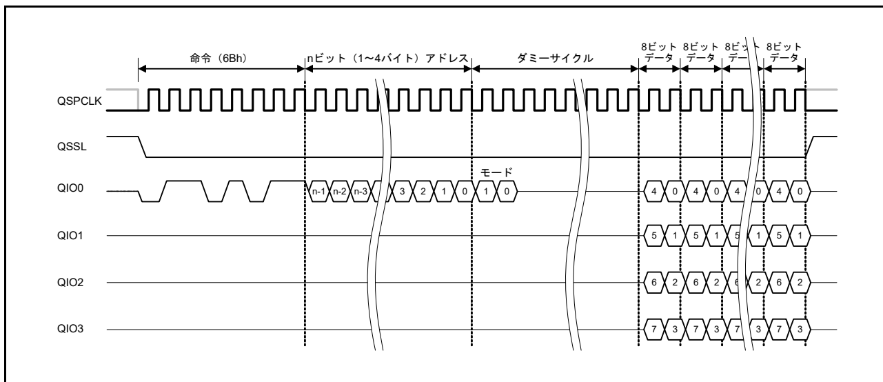
図 37.23 ファストリード Quad 出力バスサイクル
