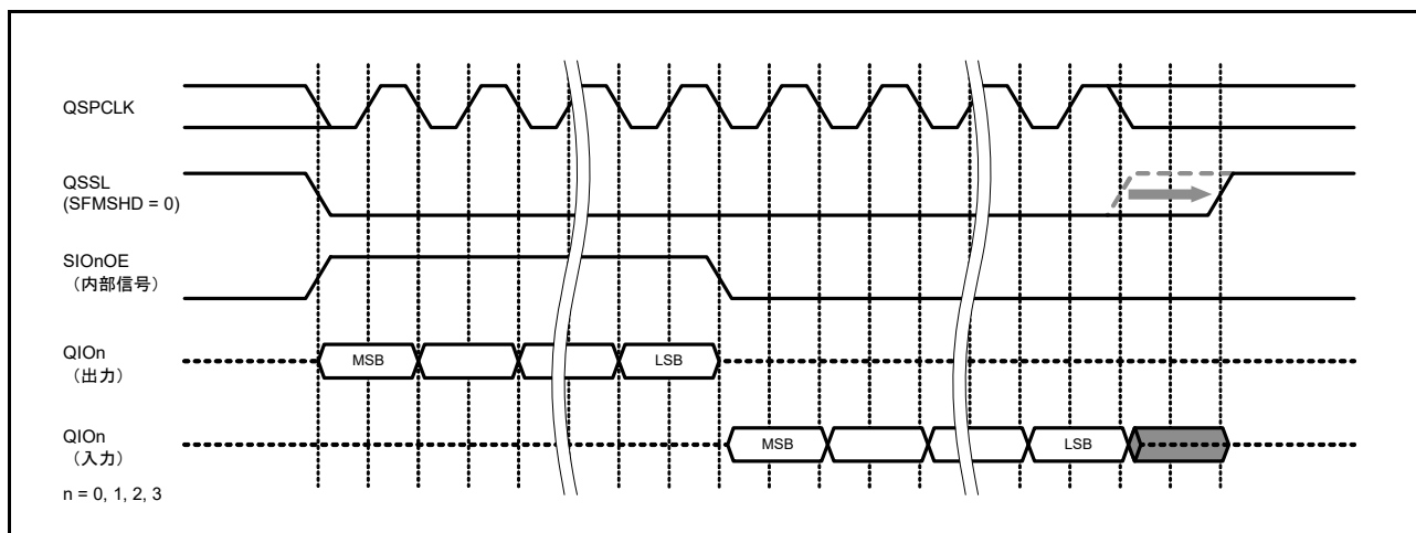
図 37.11 SFMSHD ビットを使用した QSSL 信号のホールド時間調整
