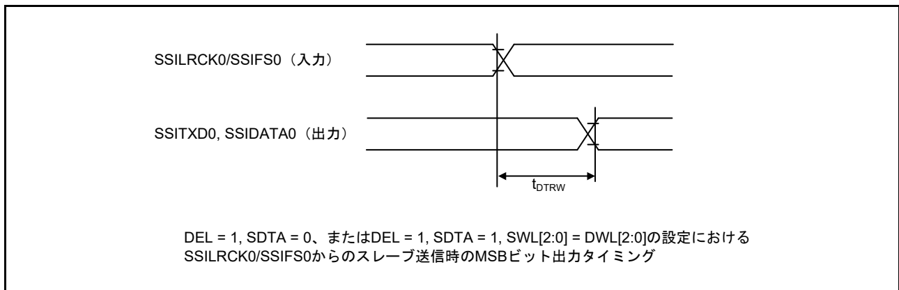
図 55.62 SSILRCK0/SSIFS0 変化時からの SSIE データ出力遅延
