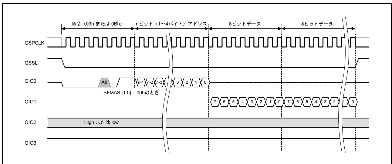
図 37.16 標準リードバスサイクル
