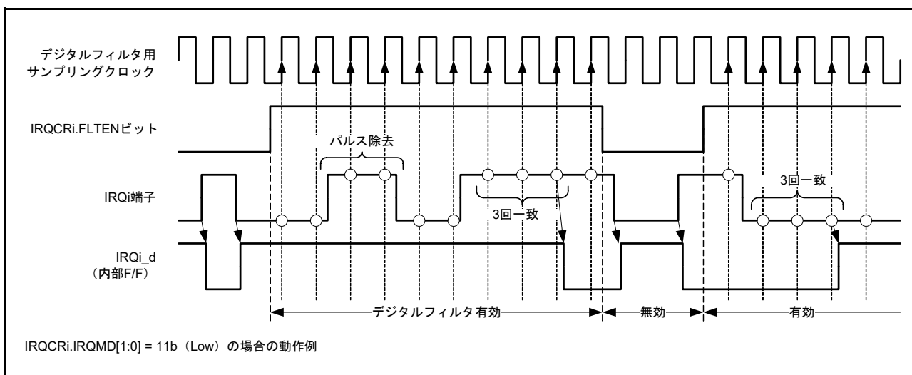
図 14.4 デジタルフィルタの動作例
