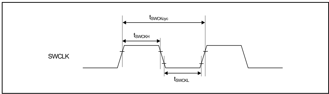
図 55.94 SWD SWCLK タイミング
