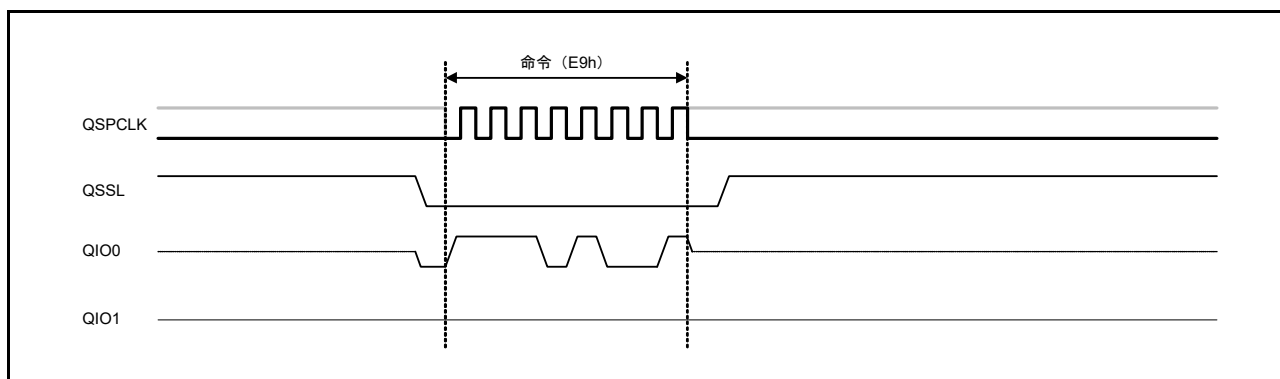
図 37.28 4 バイトモード解除バスサイクル
