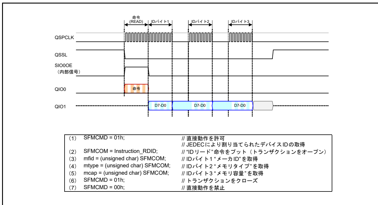
図 37.34 ID リードの直接通信タイミング例
