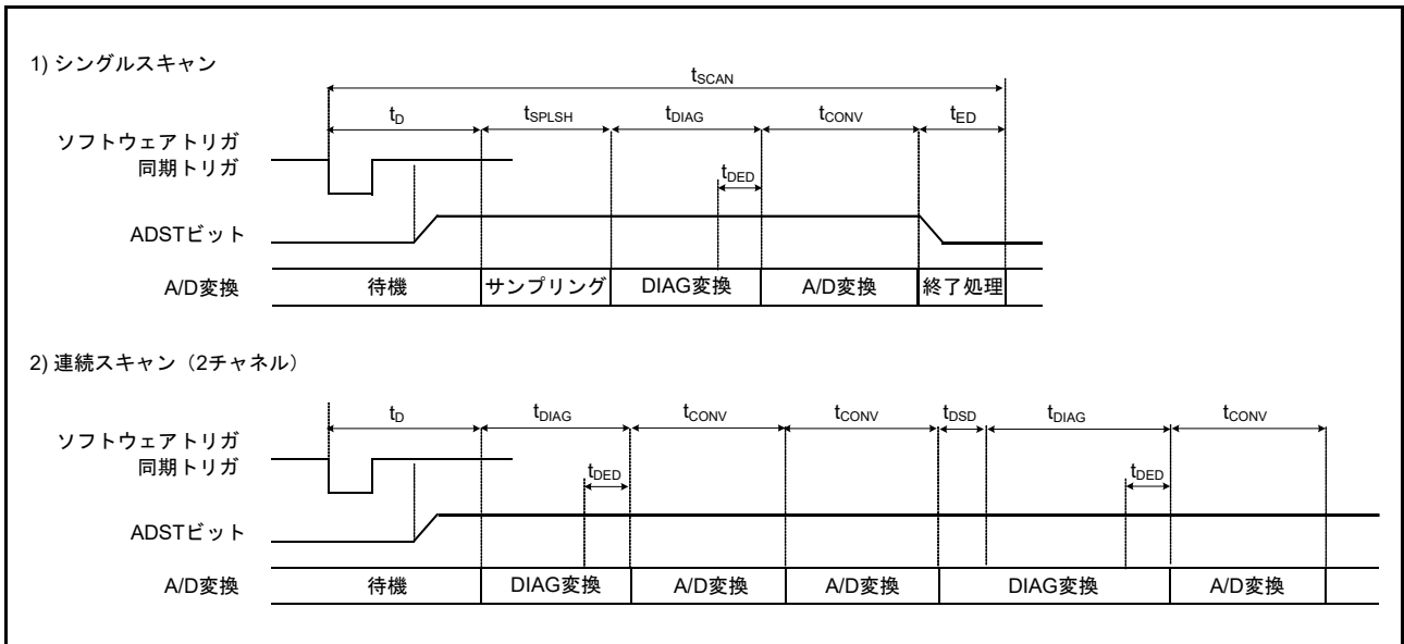
図 45.34 スキャン変換のタイミング (ソフトウェア起動または同期トリガ入力 (ELC) 起動の場合)
