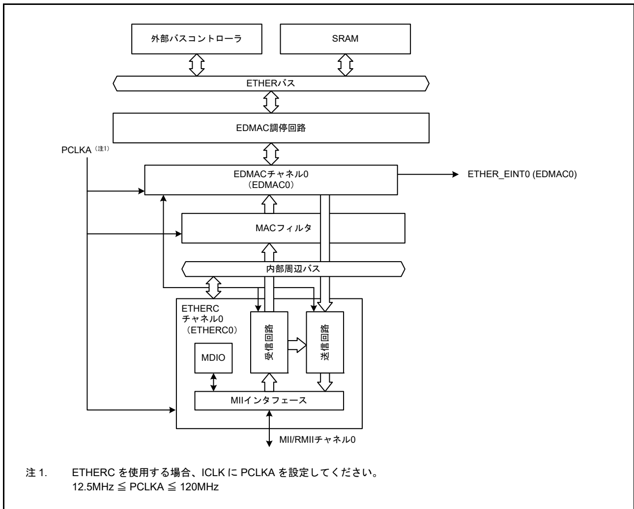
図 29.1 ETHERC の構成
