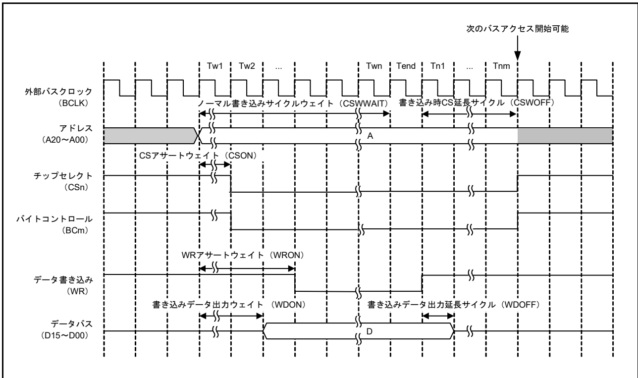
図 15.12 ノーマルライトアクセスのバスタイミング (1 ライトストローブモード) (n = 0 ~ 7 および m = 0, 1)
