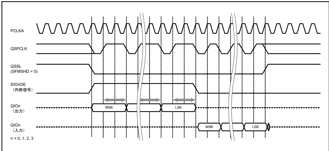
図 37.14 SFMOHW ビットを使用したシリアルデータ出力のホールド時間調整
