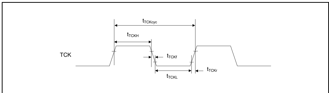
図 55.92 JTAG TCK タイミング
