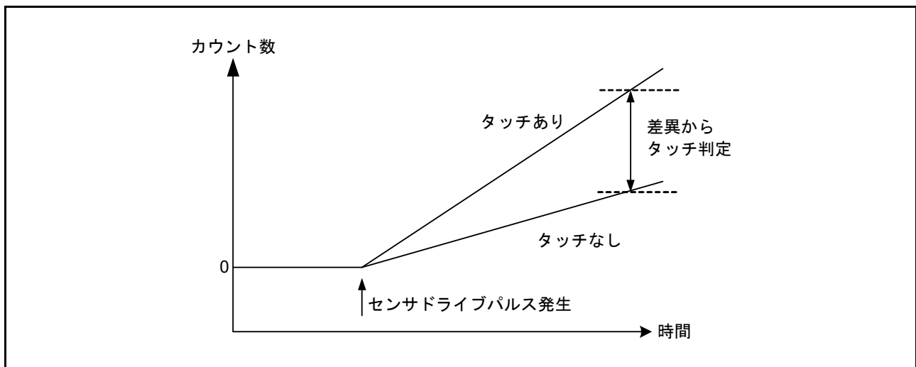
図 49.7 接触／非接触による計測値の変化
