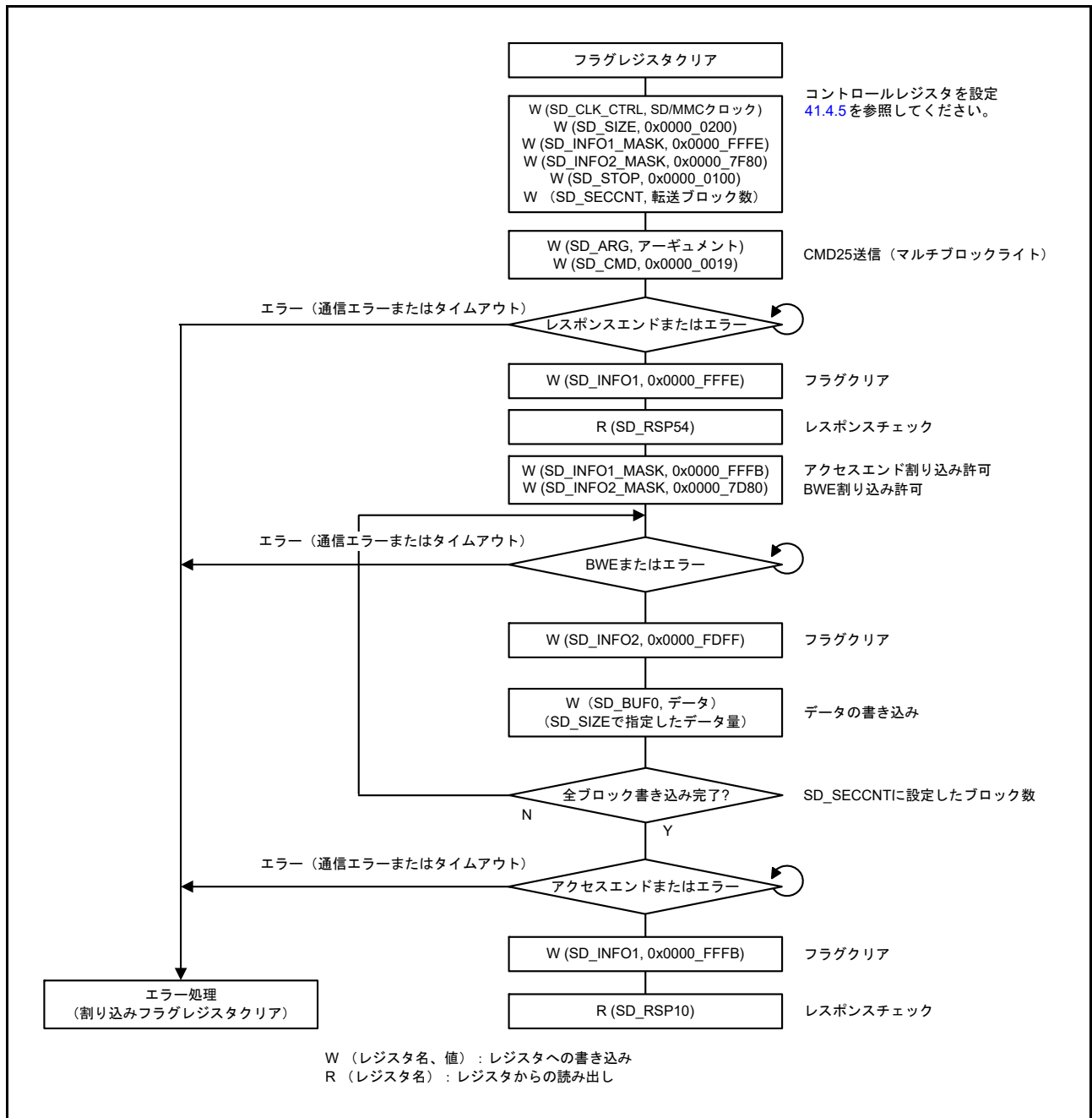
図 41.14 内蔵タイマによるマルチブロックライト動作の例
