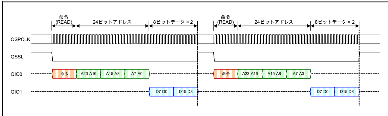
図 37.30 個々の変換に基づく連続データリード動作
