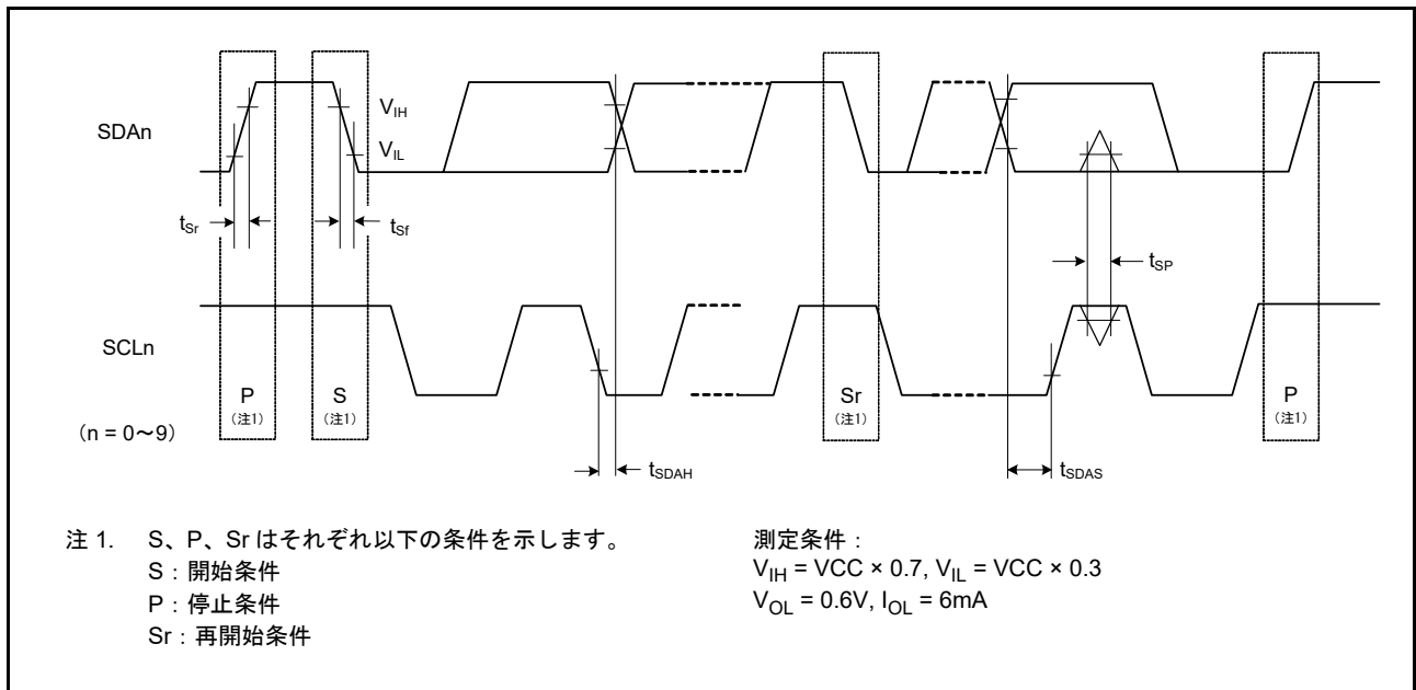
図 55.47 SCI 簡易 IIC モードタイミング
