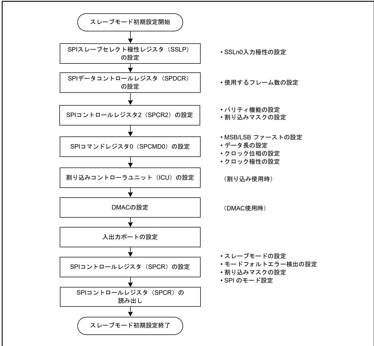
図 36.40 スレーブモード時の SPI 動作の初期化フロー例
