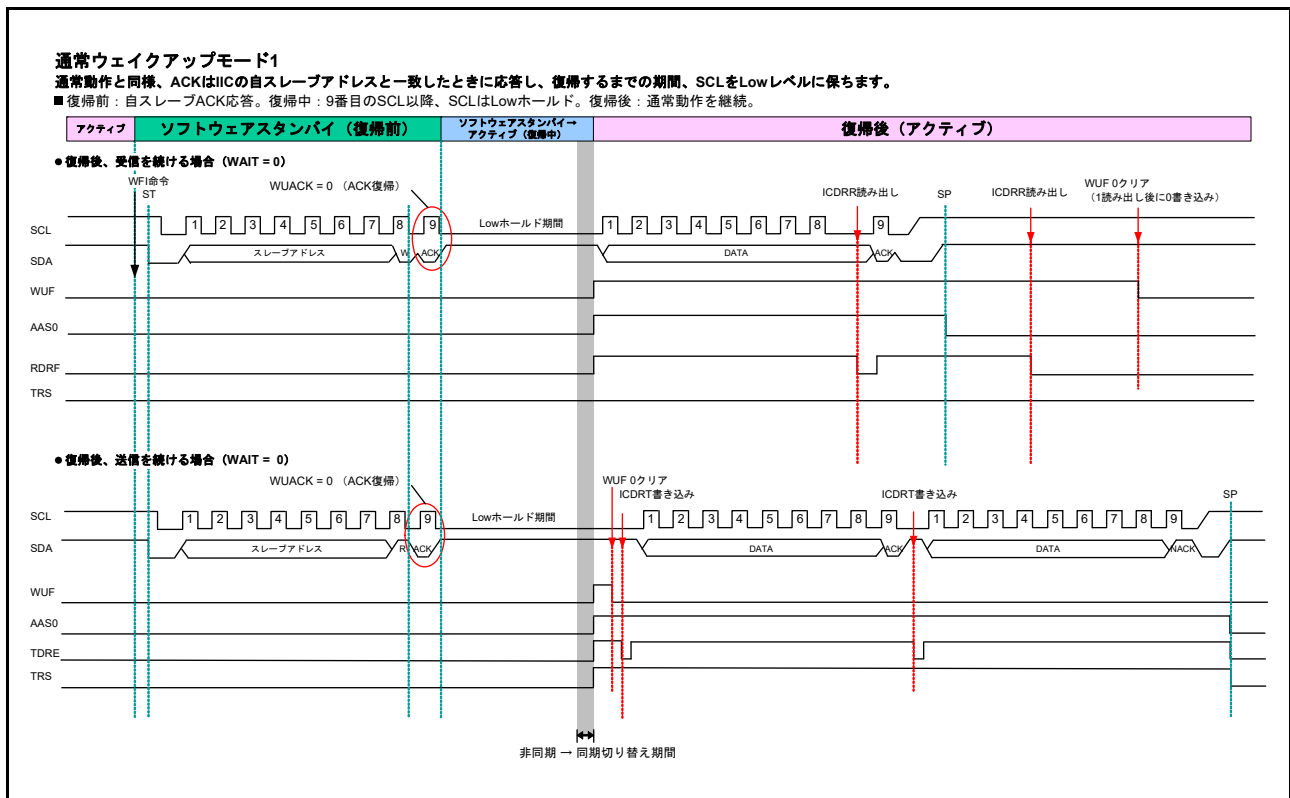
図 34.32 ノーマルウェイクアップモード1のタイミング
