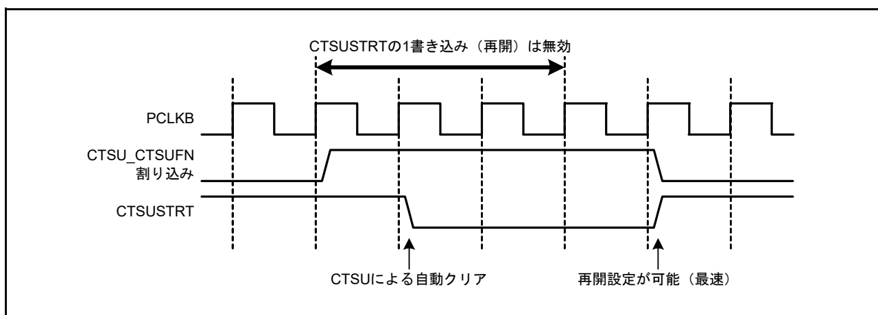
図 49.21 再開時の注意事項
