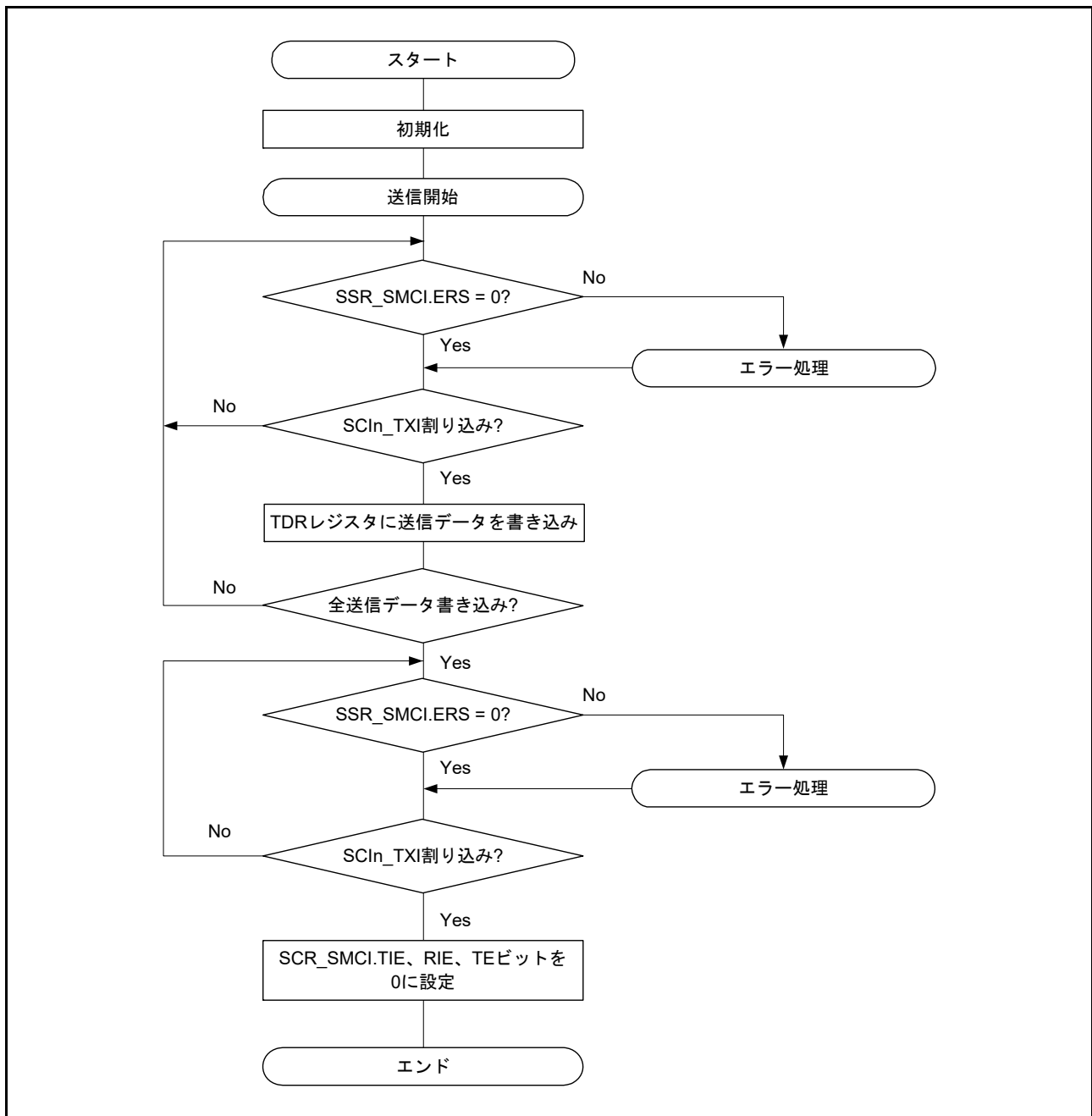
図 32.54 スマートカードインタフェース送信のフローチャート例
