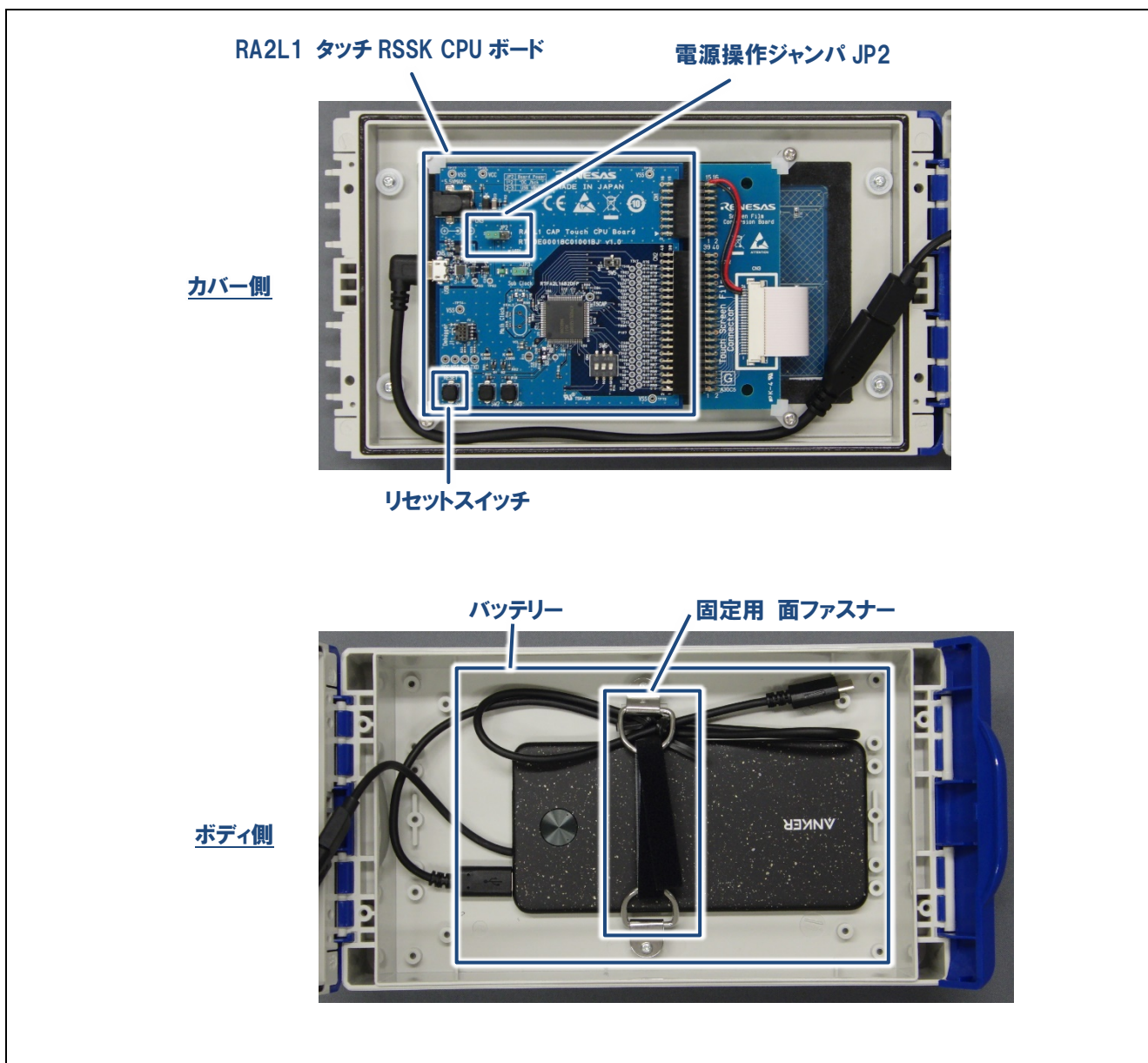
図 2-3 内部構成
