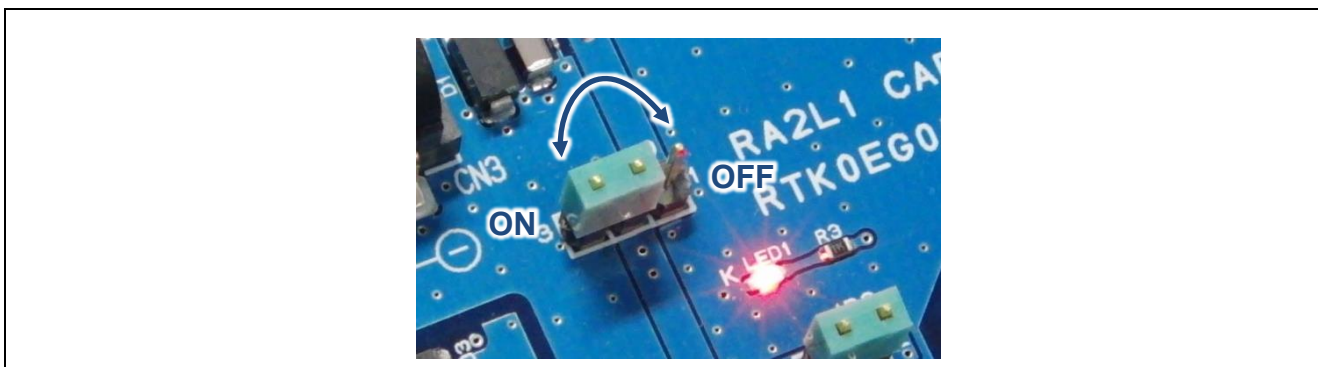
図 3-4 CPU ボードのジャンパ電源操作
