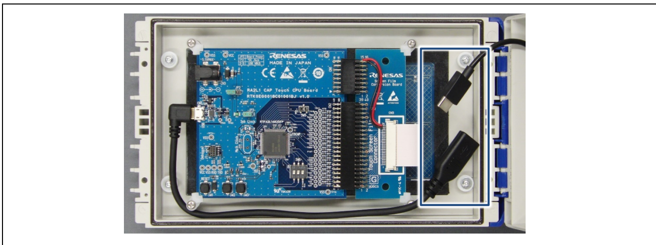
図 3-5 USB ケーブル中間コネクタの電源操作
