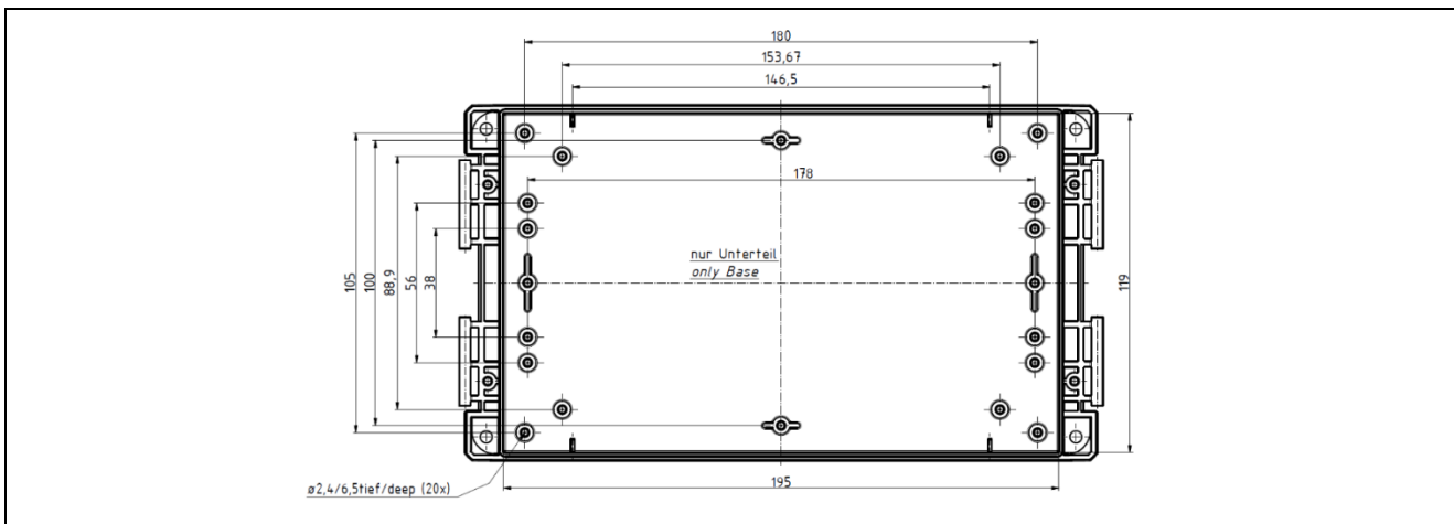
図 4-2 ボディ内寸
