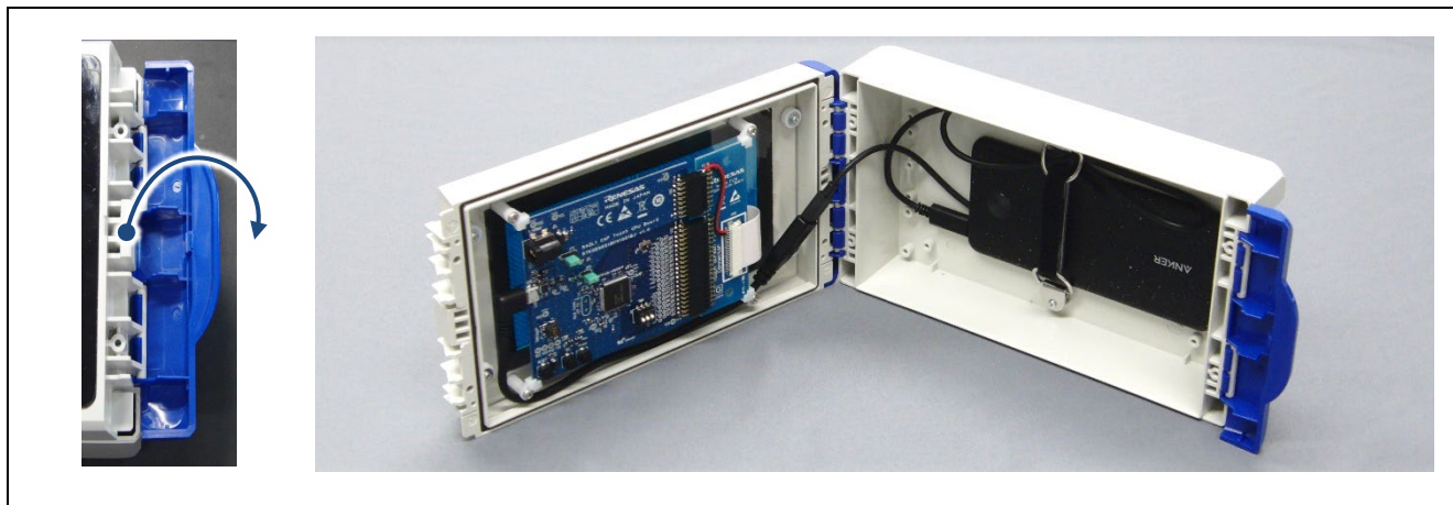
図 3-1 カバーの開け方
