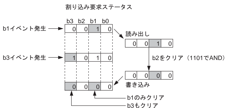
図 28.3 割り込み要求ステータスクリア例
