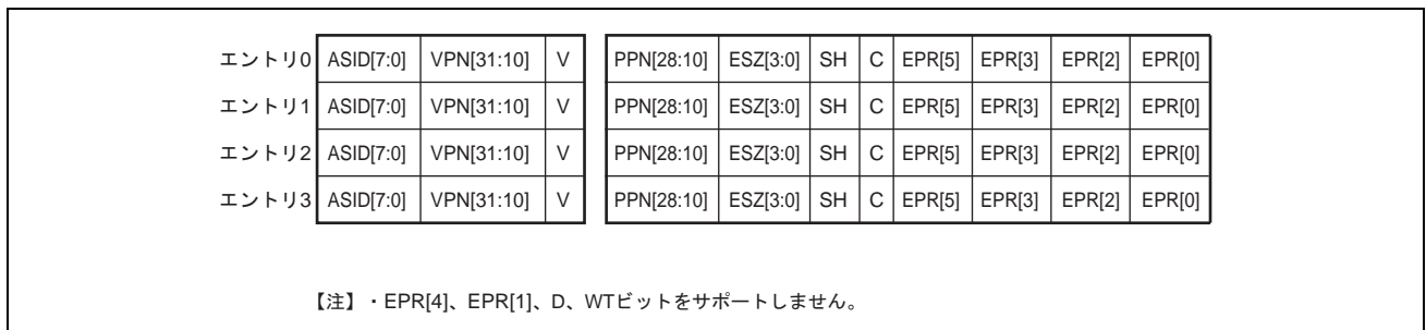
図 7.13 ITLB の構成 (TLB 拡張モード)
