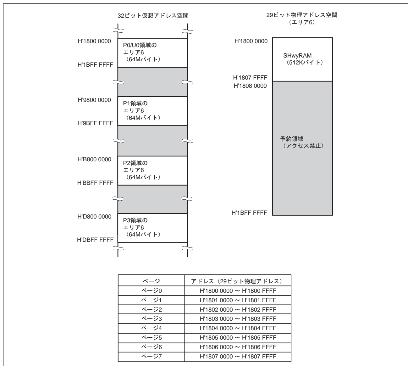
図 13.3 SH74593 のアドレス空間
