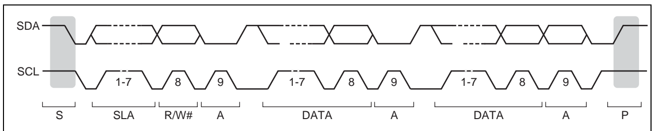
図 25.4 I 2 C バスタイミング
