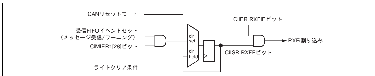
図 26.24 CAN i 受信 FIFO 割り込み[RXF i ]のブロック図
