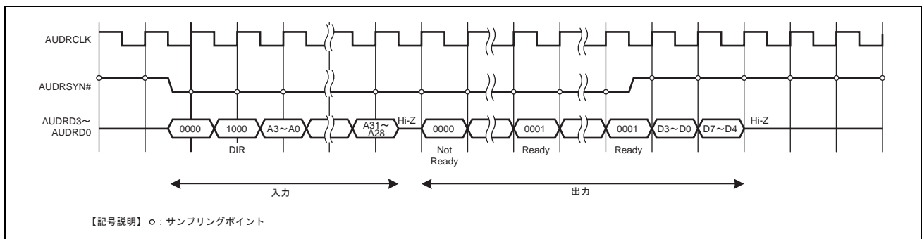
図 36.5 リード動作例 (バイトリード)
