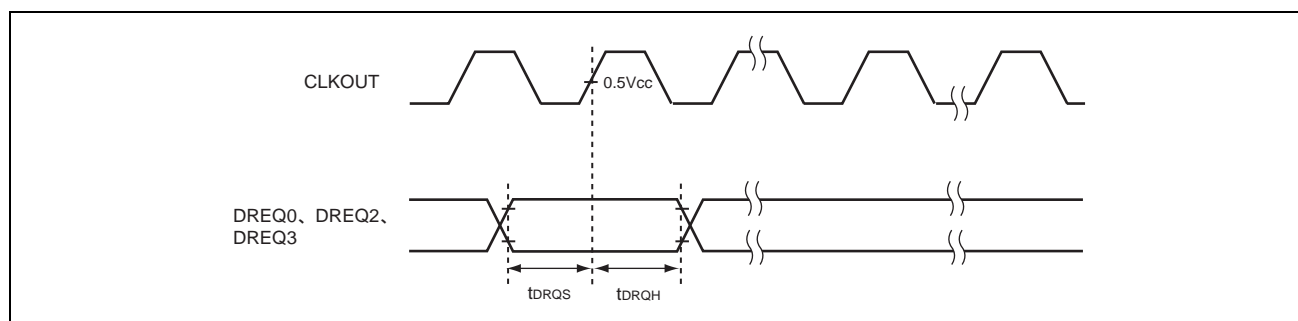
図 38.12 DMAC タイミグ
