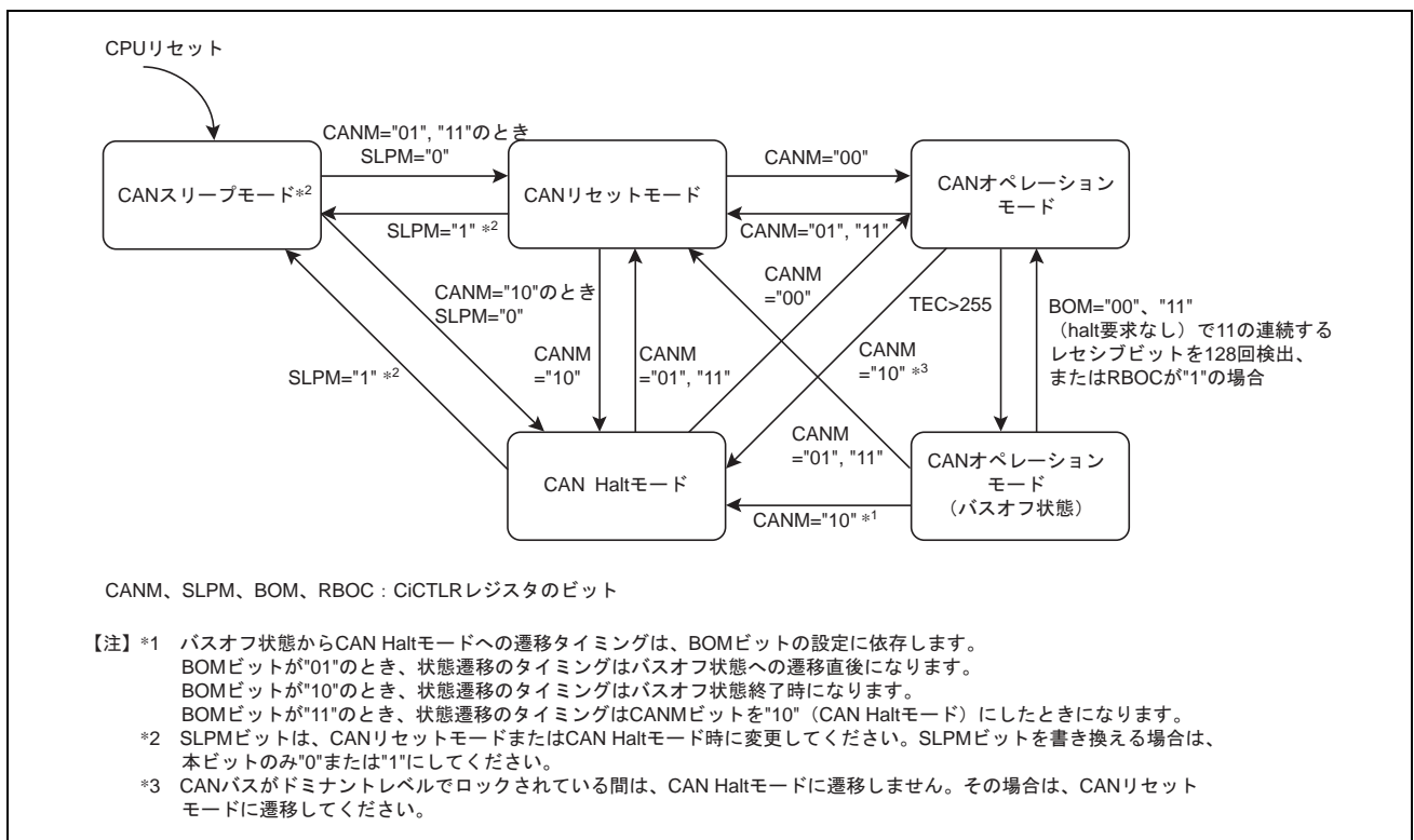
図 26.9 CAN 動作モード間の遷移 (i=0~3)
