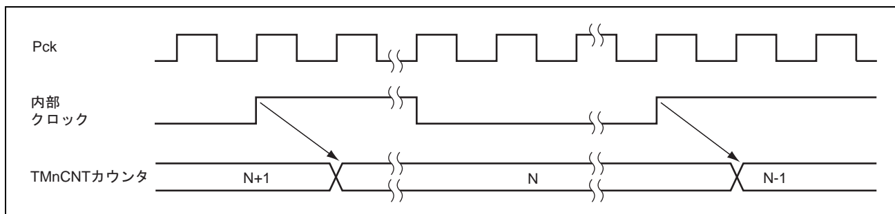
図 22.4 内部クロック動作時のカウンタタイミング
