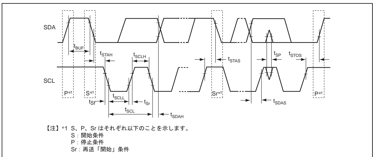
図 38.24 IIC3 モジュール入出力タイミング
