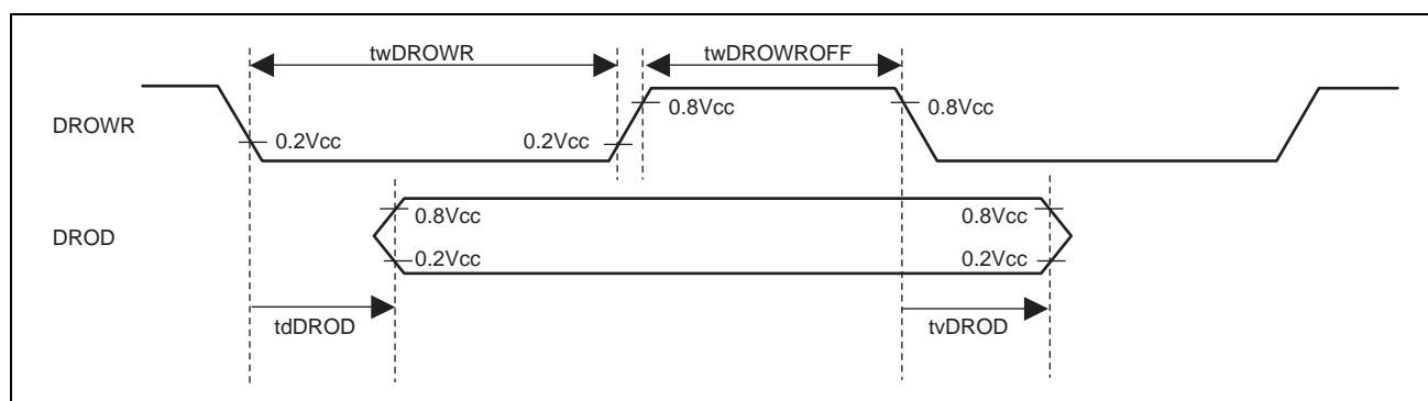
図 38.29 "L"アクティブ選択時のストロブ極性
