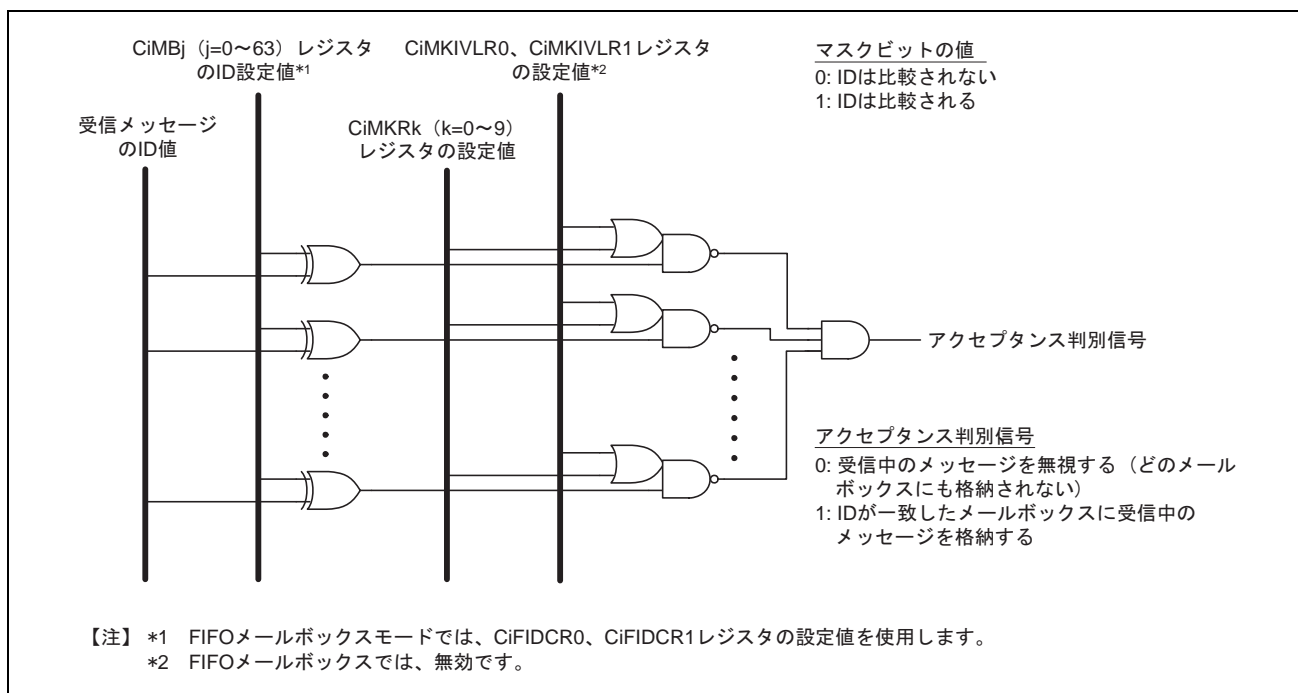
図 26.17 アクセプタンスフィルタ処理 ( i=0\sim 3 )
