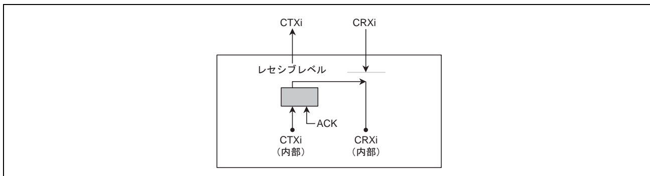
図 26.8 セルフテストモード 1 選択時の接続
