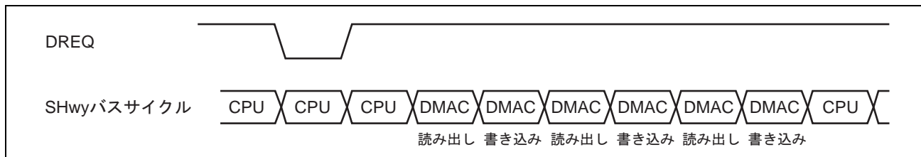
図 20.4 バーストモードでの DMA 転送例 (DREQ 信号立ち下がリエッジ有効設定時)
