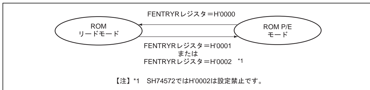
図 12.7 FCU のモード遷移図 (ROM 関連)
