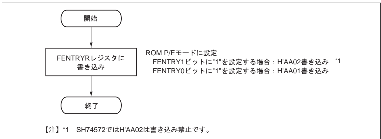
図 12.9 ROM P/E モード移行フロー
