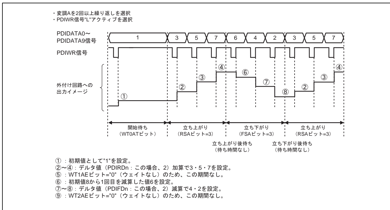
図 30.18 各変調の初期値・デルタ値反映タイミング (待ち時間なし)
