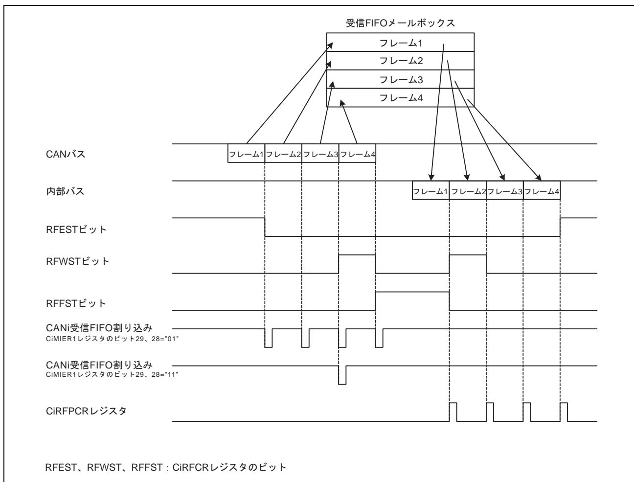
図 26.2 受信 FIFO メールボックスの動作(CiMIER1 レジスタのビット 29、28 が"01"または"11") (i=0~3)
