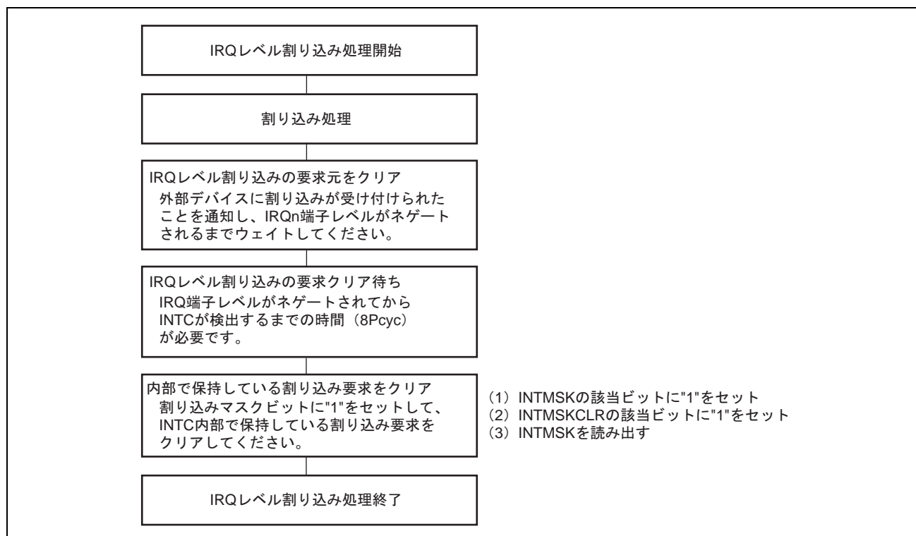
図 15.9 割り込み処理ルーチンの例
