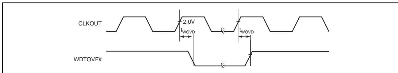
図 38.16 WDT タイミグ
