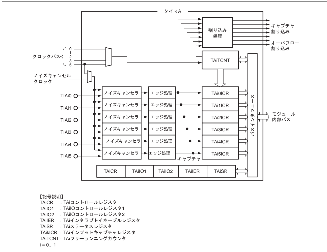
図 21.7 タイマ A のブロック図
