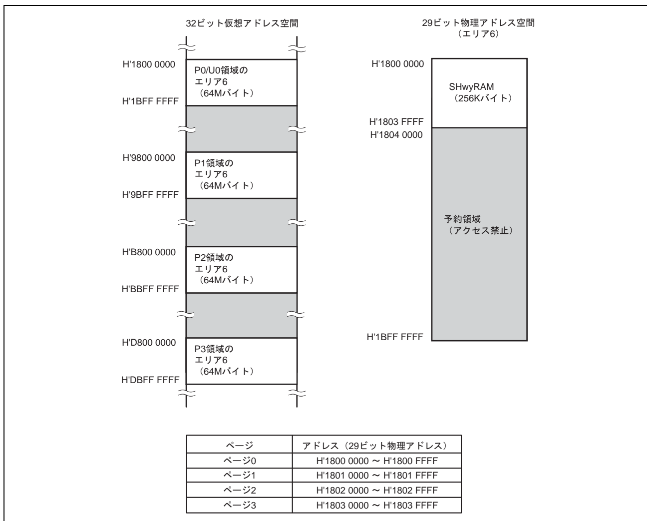
図 13.2 SH74572 のアドレス空間
