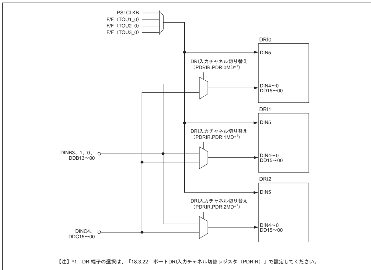
図 28.12 DRI 端子と DRI モジュール端子との接続イメージ
