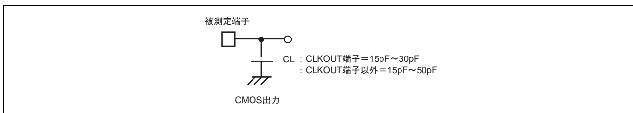
図 38.1 出力スイッチング特性測定回路
