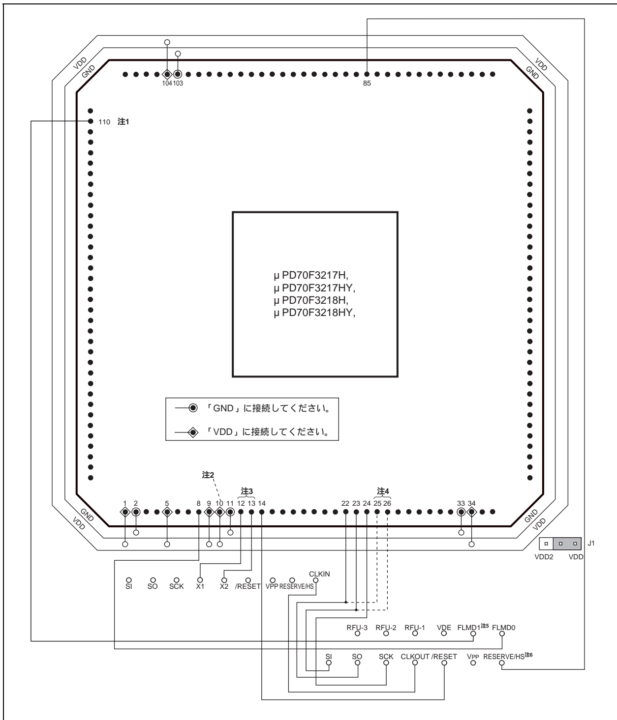
★ 図26 - 6 V850ES/KJ1フラッシュ書き込み用アダプタ (FA-144GJ-UEN-A) の配線例 (1/2)
