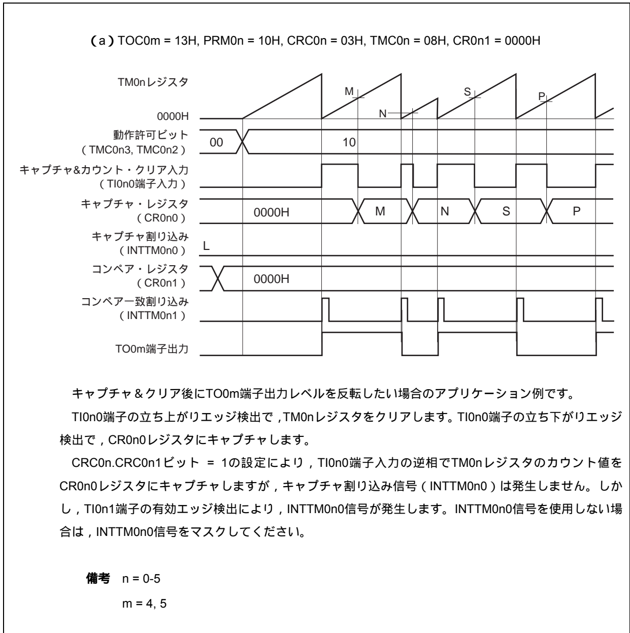
図8 - 18 TI0n0端子の有効エッジ入力によるクリア&スタート・モードのタイミング例 (CR0n0レジスタ：キャプチャ・レジスタ/CR0n1レジスタ：コンペア・レジスタ) (1/2)
