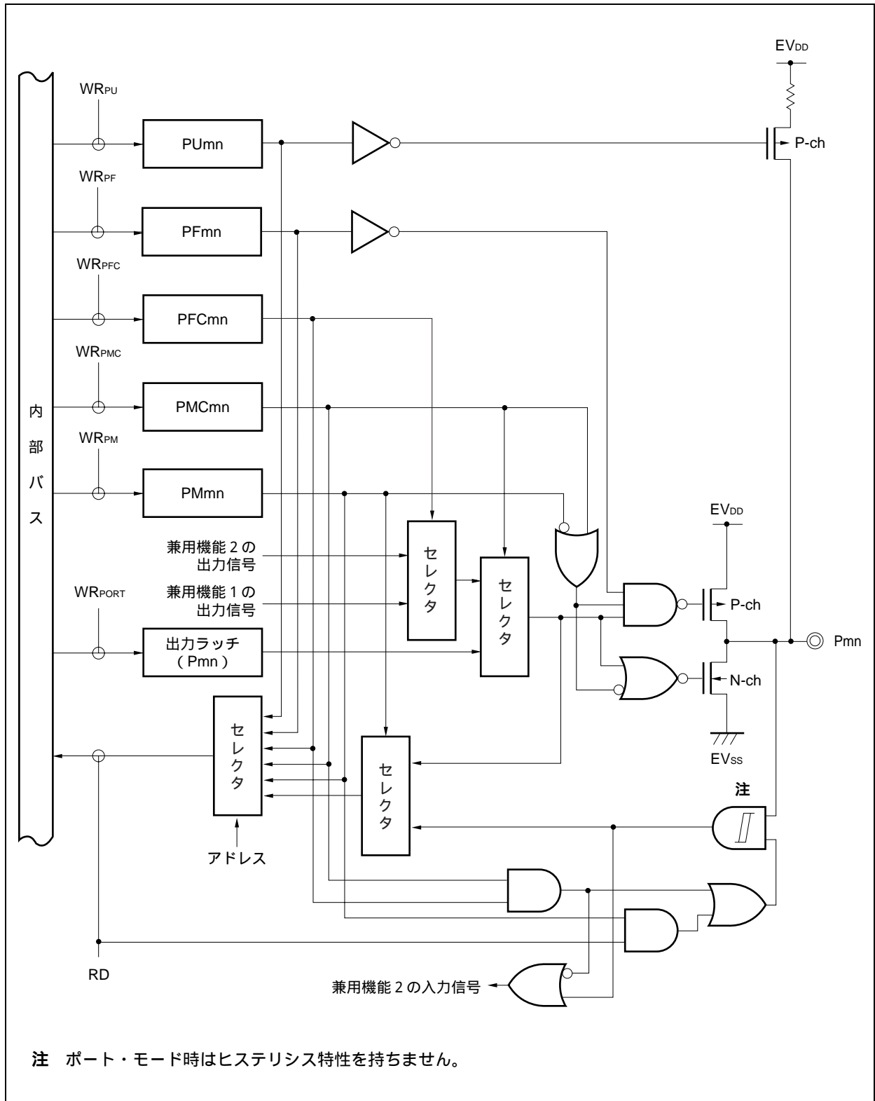
図4 - 25 タイプG-6のブロック図
