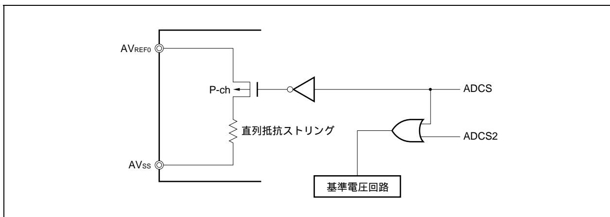
図14 - 5 スタンバイ・モード時の消費電力を低減させる方法例
