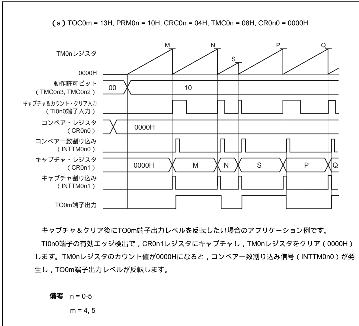
図8 - 16 TI0n0端子の有効エッジ入力によるクリア&スタート・モードのタイミング例 (CR0n0レジスタ：コンペア・レジスタ/CR0n1レジスタ：キャプチャ・レジスタ) (1/2)
