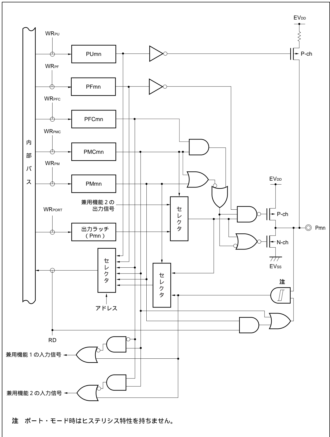
図4-24 タイプG-5のブロック図
