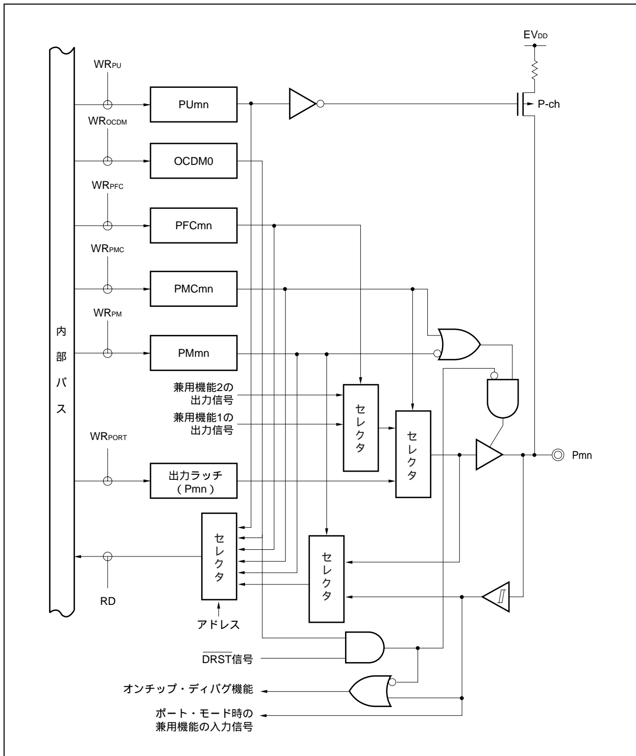
図4 - 34 タイプO-3のブロック図
