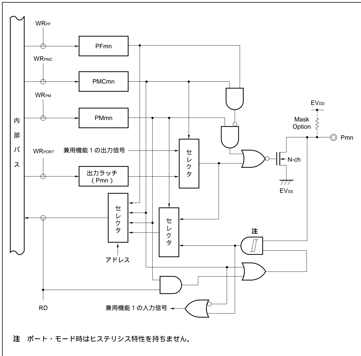
図4 - 31 タイプKのブロック図
