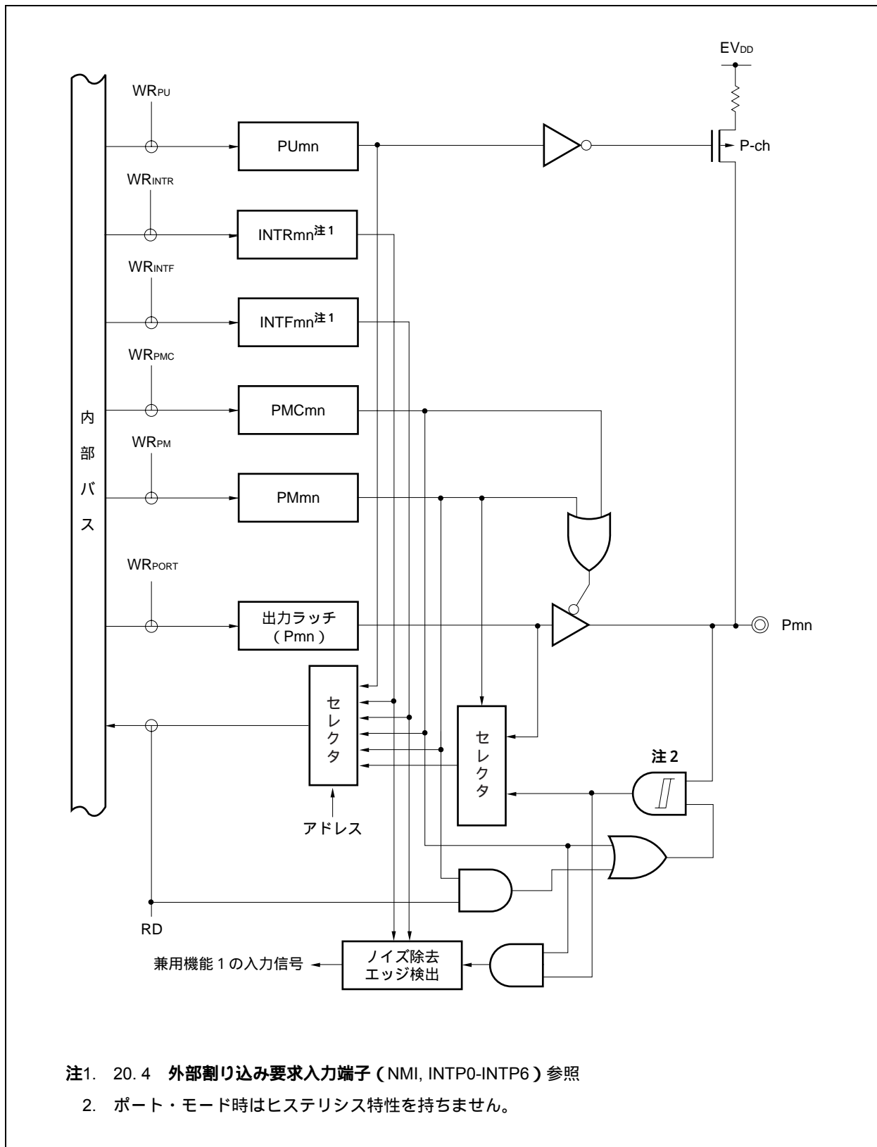
図4-28 タイプH-1のブロック図
