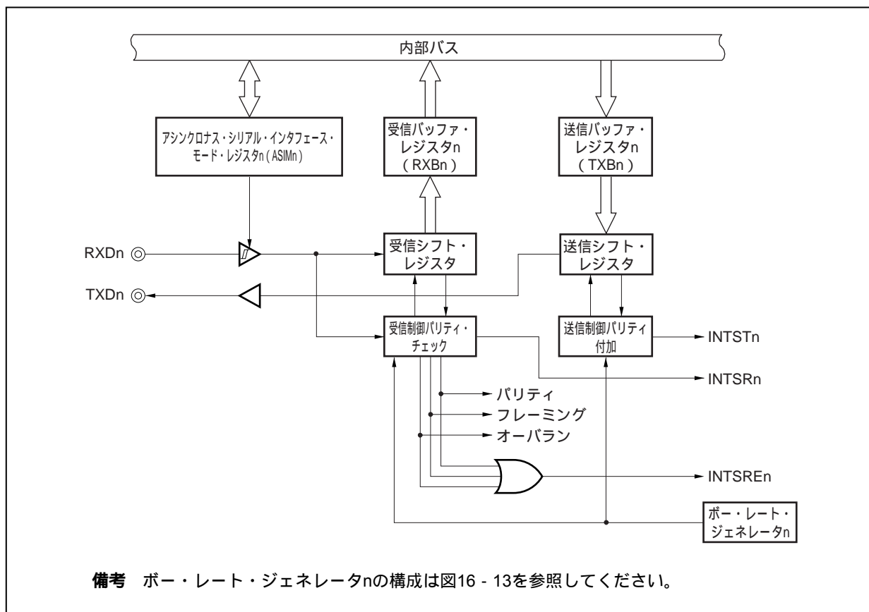
図16 - 2 UART n のブロック図
