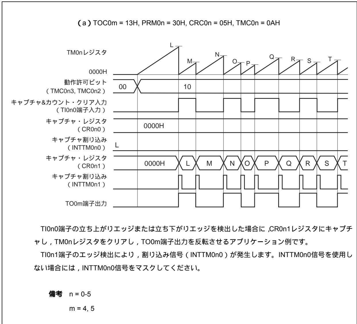
図8 - 20 TI0n0端子の有効エッジ入力によるクリア&スタート・モードのタイミング例 (CR0n0レジスタ：キャプチャ・レジスタ/CR0n1レジスタ：キャプチャ・レジスタ) (1/3)
