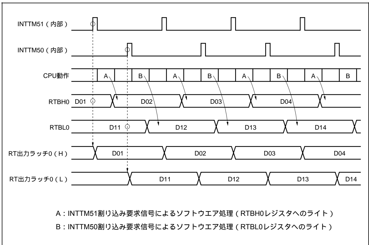
図13 - 2 RTO0の動作タイミング例 (EXTR0ビット = 0, BYTE0ビット = 0の場合)
