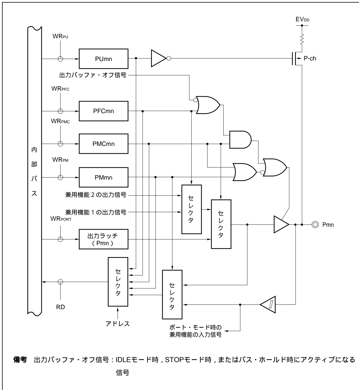
図4 - 14 タイプE-3のブロック図
