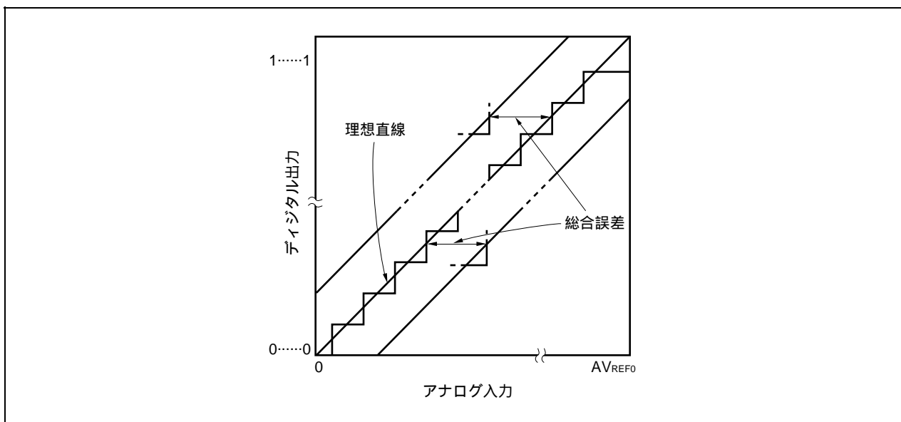
図14 - 10 総合誤差
