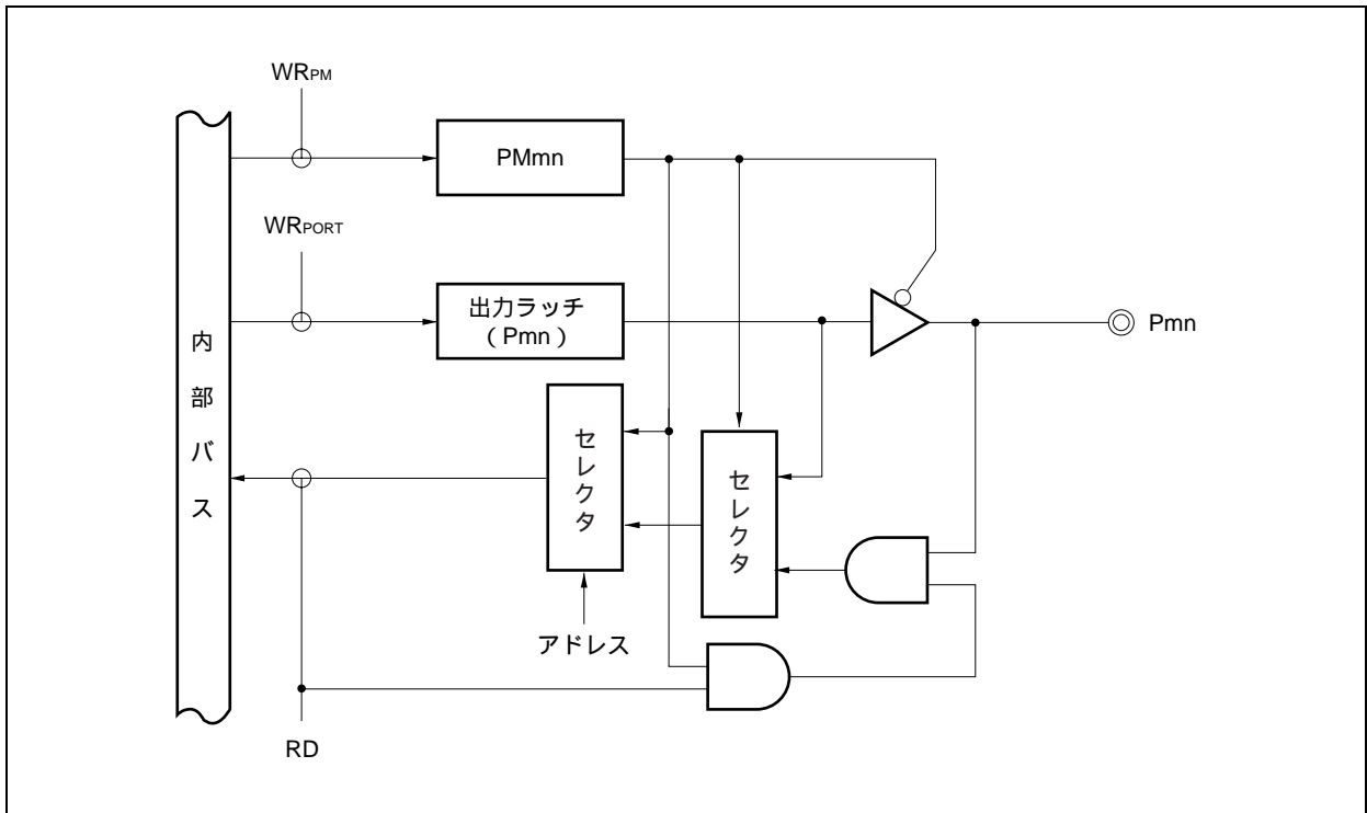
図4 - 4 タイプB-1のブロック図
