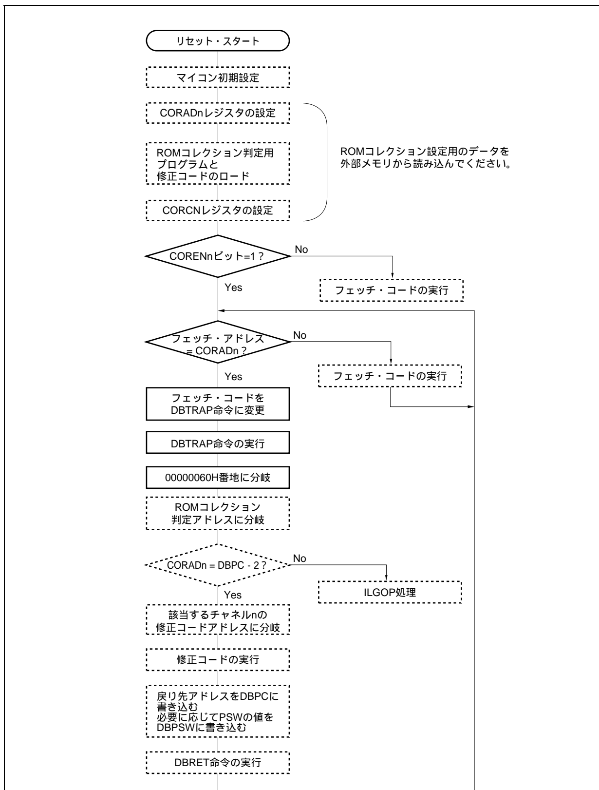
図25 - 2 ROMコレクションの動作とプログラムの流れ
