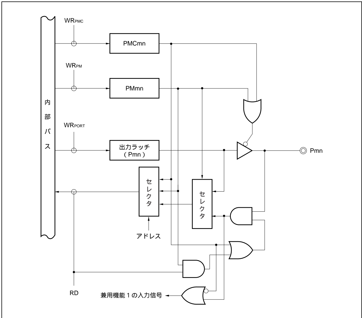
図4 - 5 タイプC-1のブロック図
