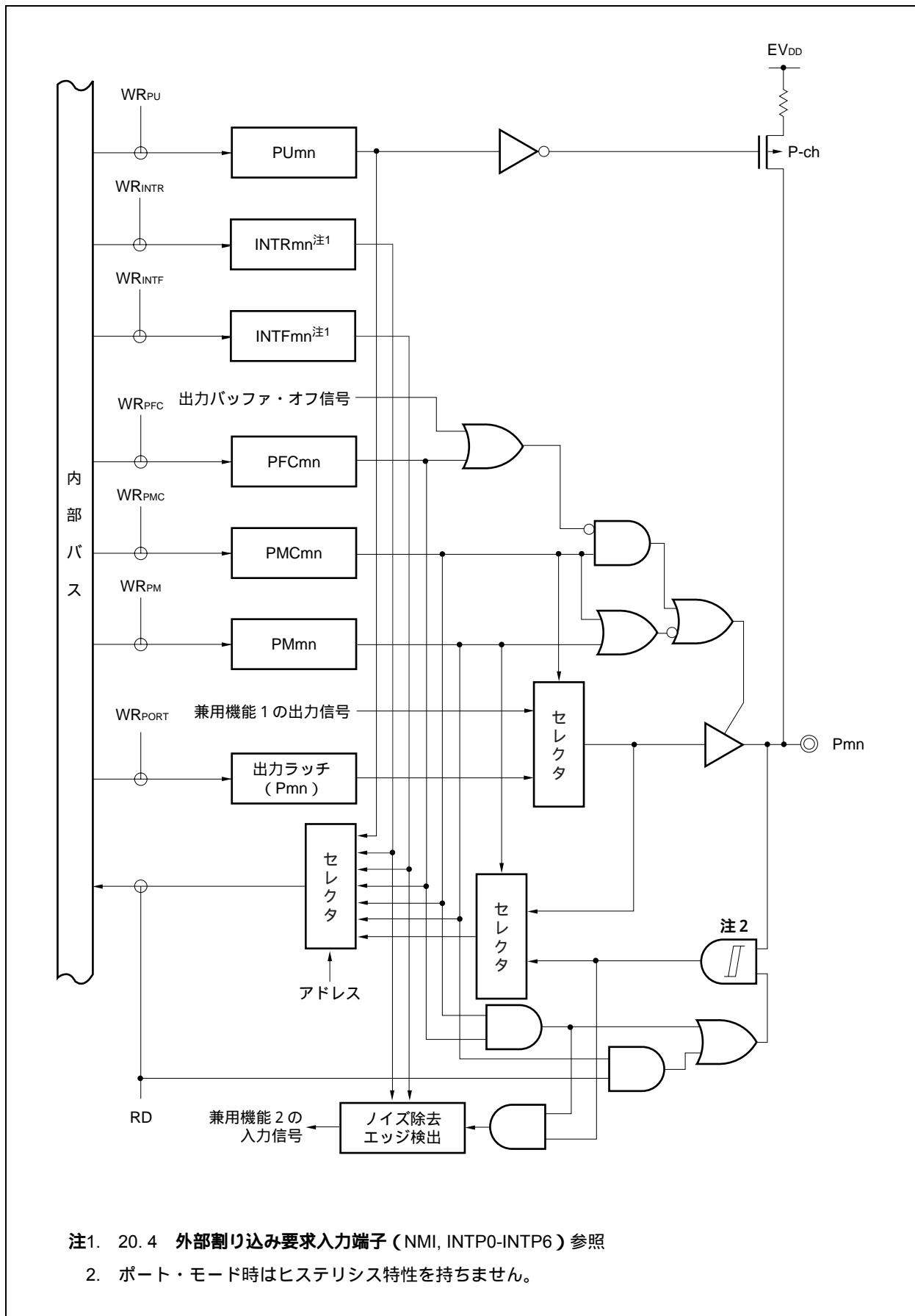
図4-29 タイプH-2のブロック図
