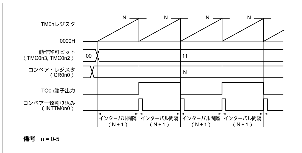
図8 - 7 方形波出力動作の基本タイミング例
