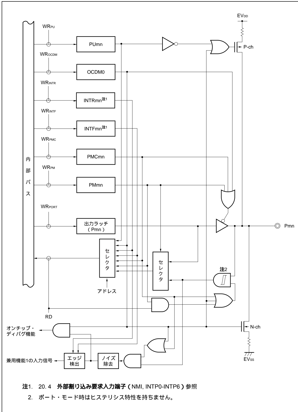
図4 - 32 タイプO-1のブロック図
