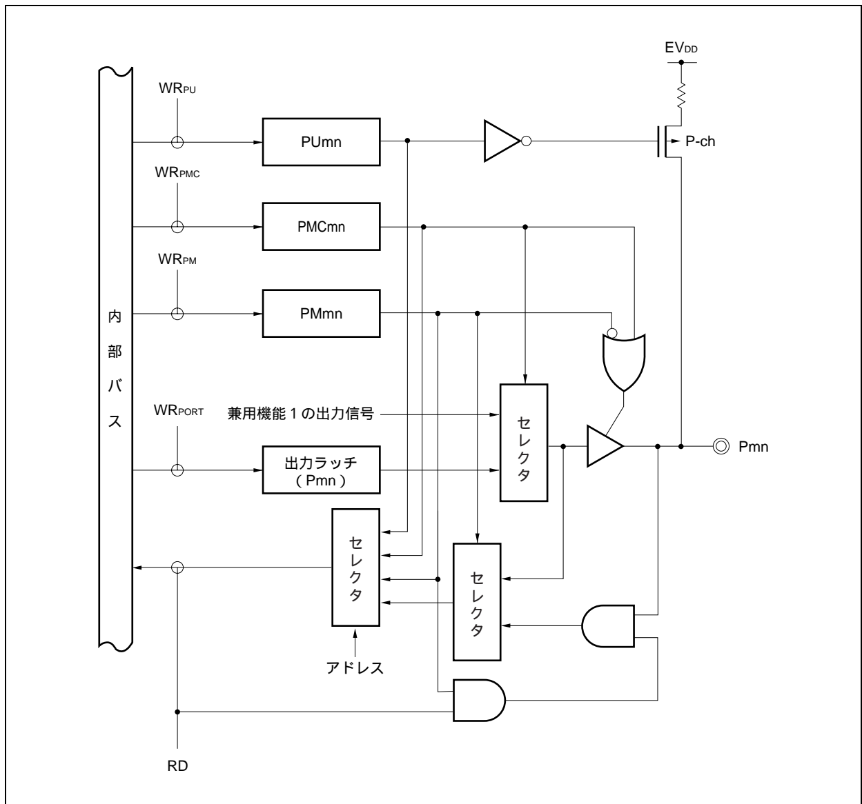
図4-11 タイプD-2のブロック図
