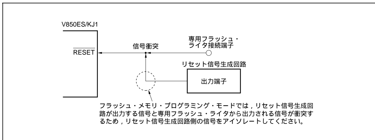
図27-9 信号の衝突（RESET端子）
