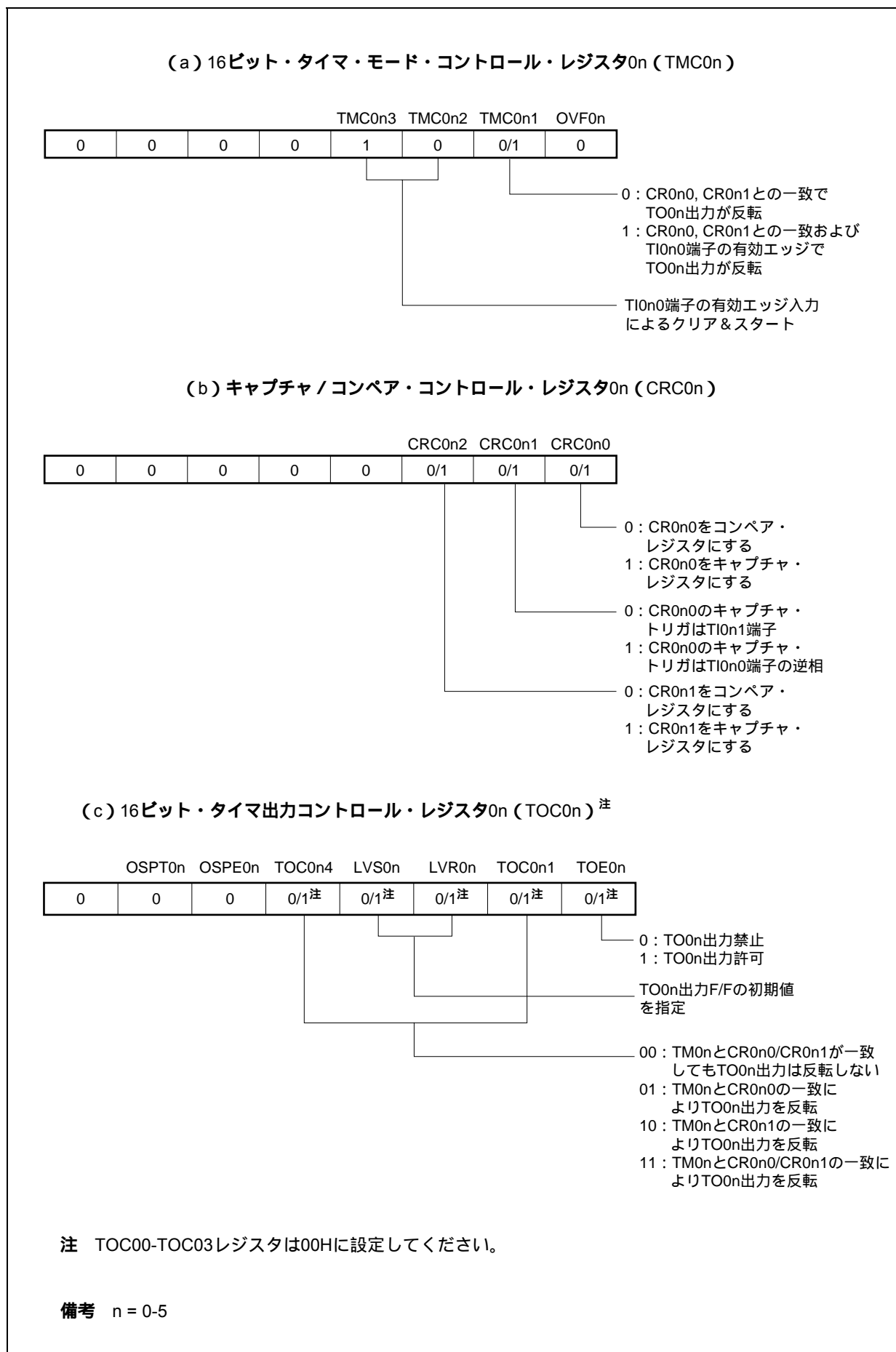
図8 - 21 TI0n0端子の有効エッジ入力によるクリア&スタート・モード動作時のレジスタ設定内容例 (1/2)
