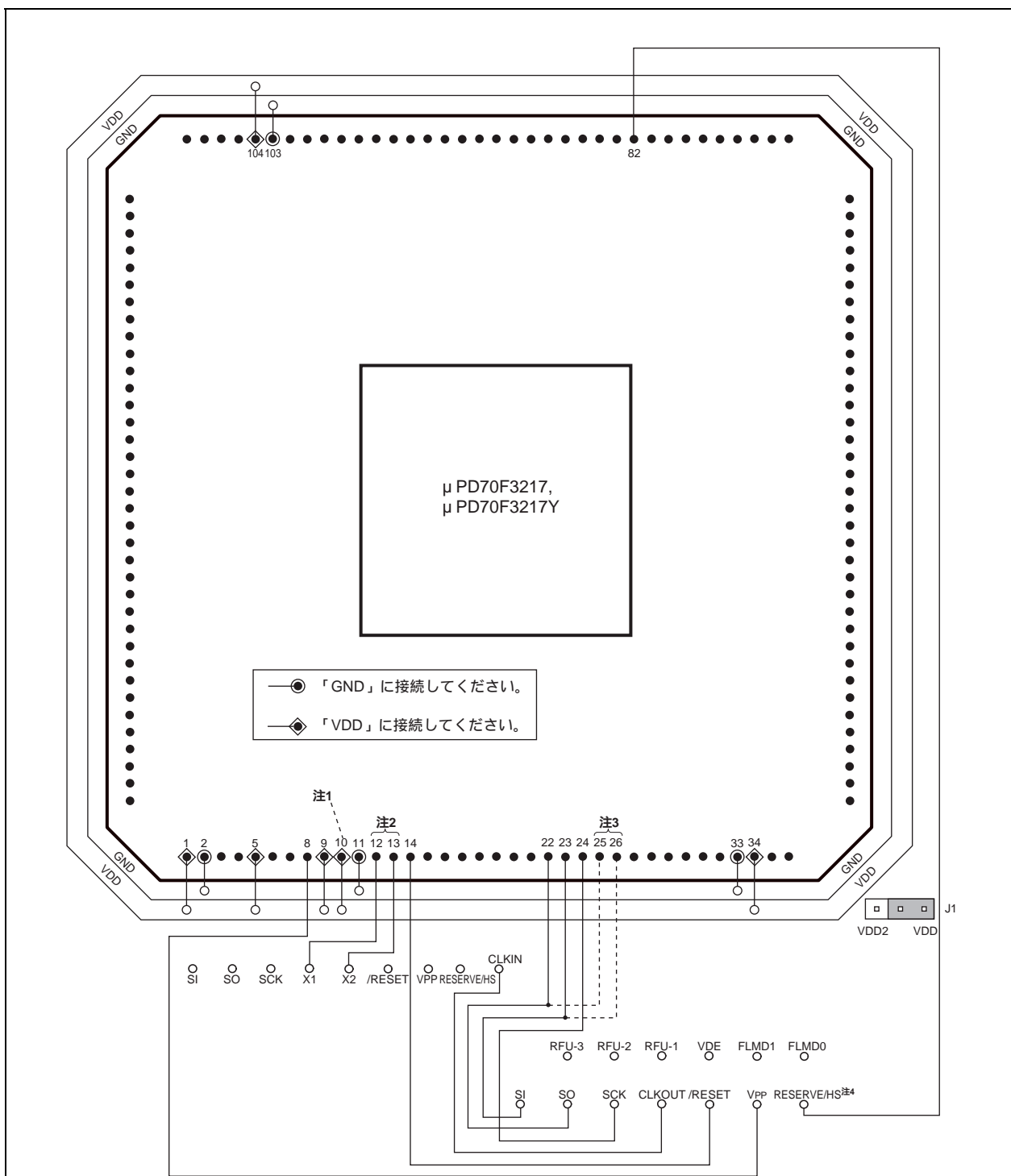
★ 図27 - 1 V850ES/KJ1フラッシュ書き込み用アダプタ (FA-144GJ-UEN-A) の配線例 (1/2)
