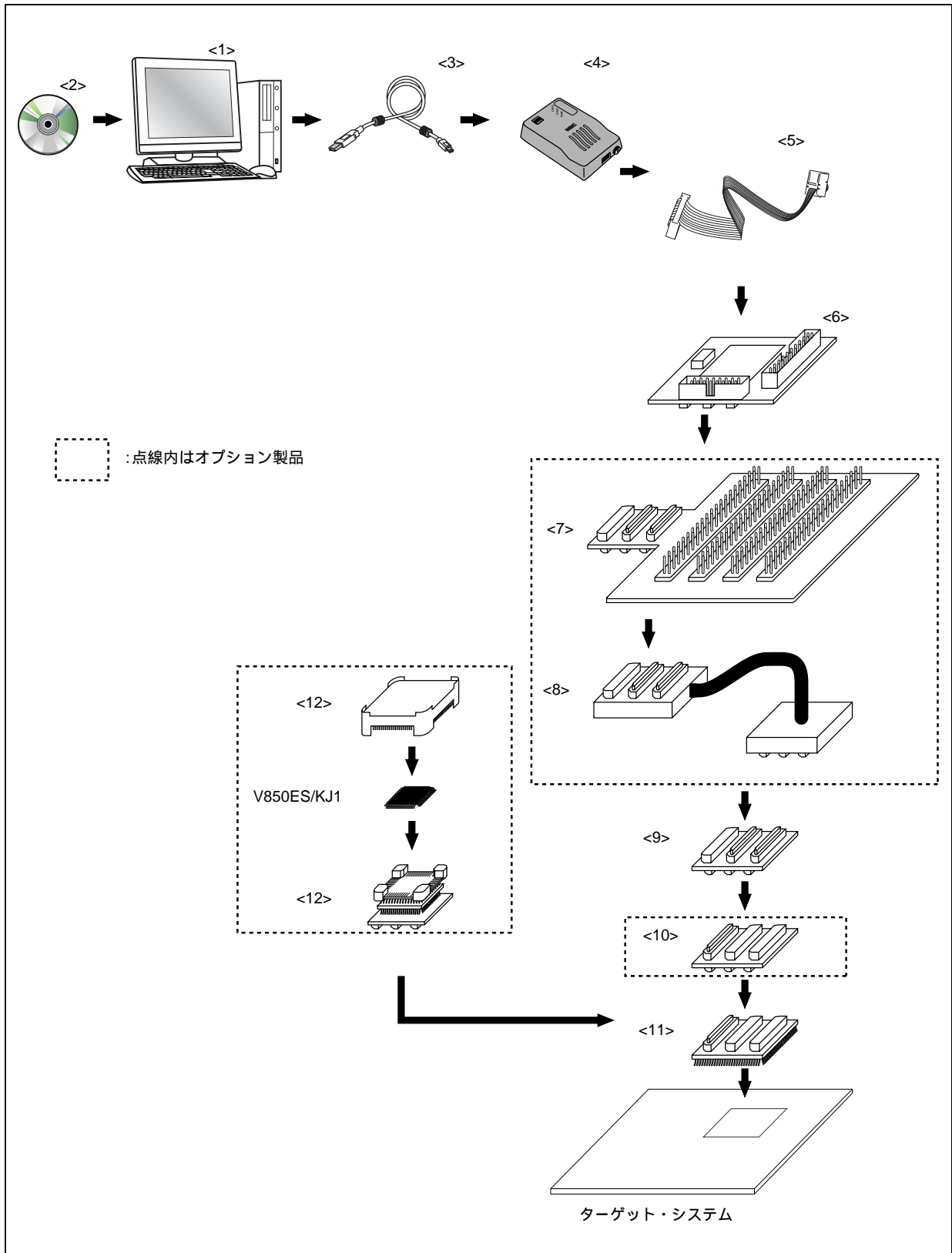
図A-4 QB-V850ESKX1-DAを使用したシステム構成(オプション製品を使用する場合)
