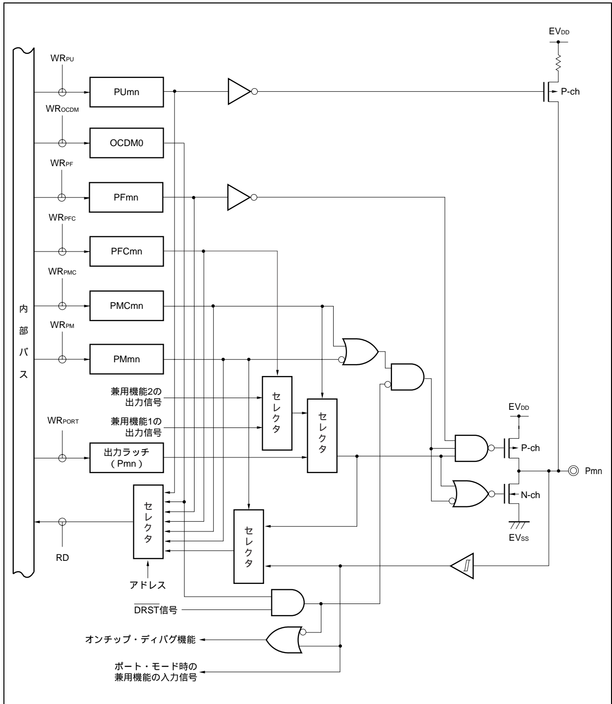
図4 - 33 タイプO-2のブロック図
