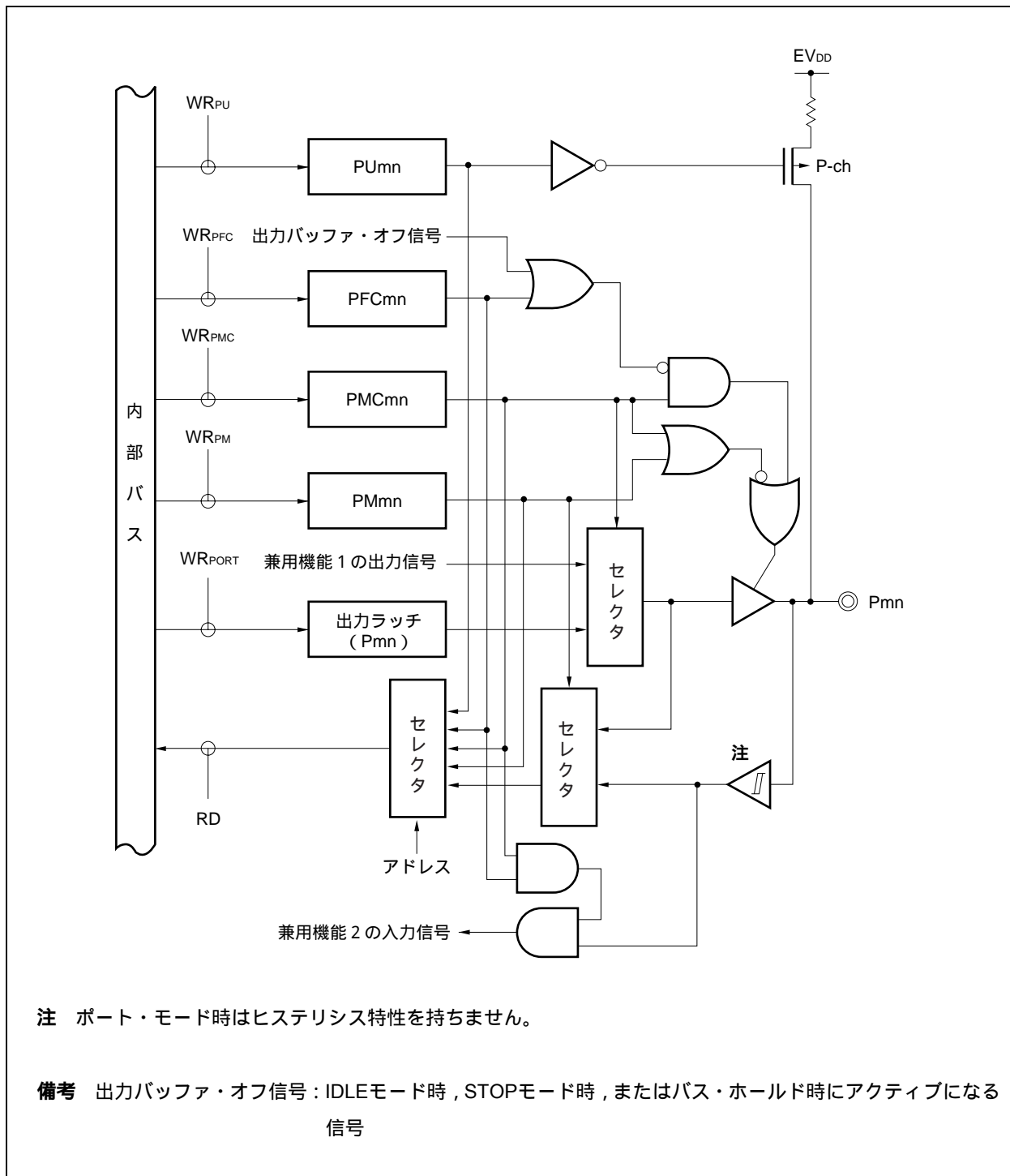
図4 - 13 タイプE-2のブロック図
