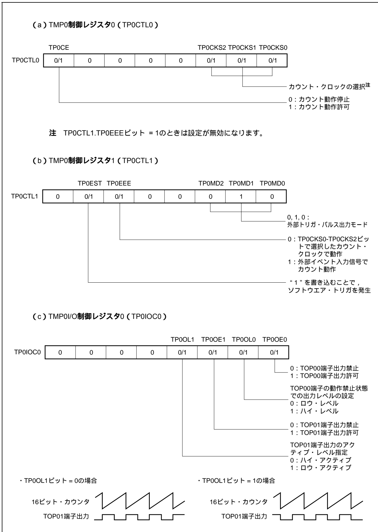
図7-18 外部トリガ・パルス出力モード動作時のレジスタ設定内容 (1/2)
