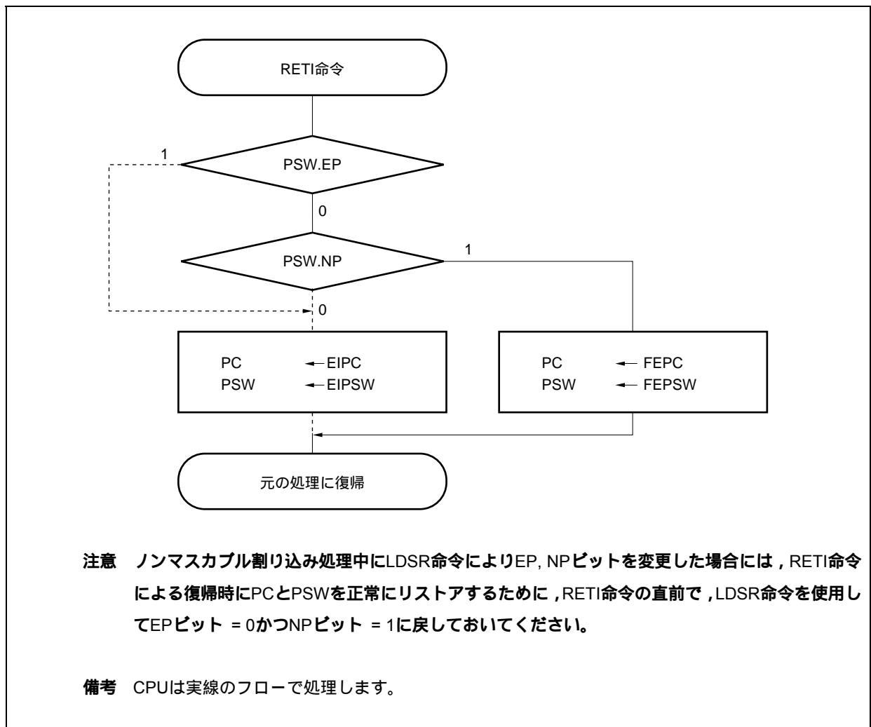
図20 - 3 RETI命令の処理形態
