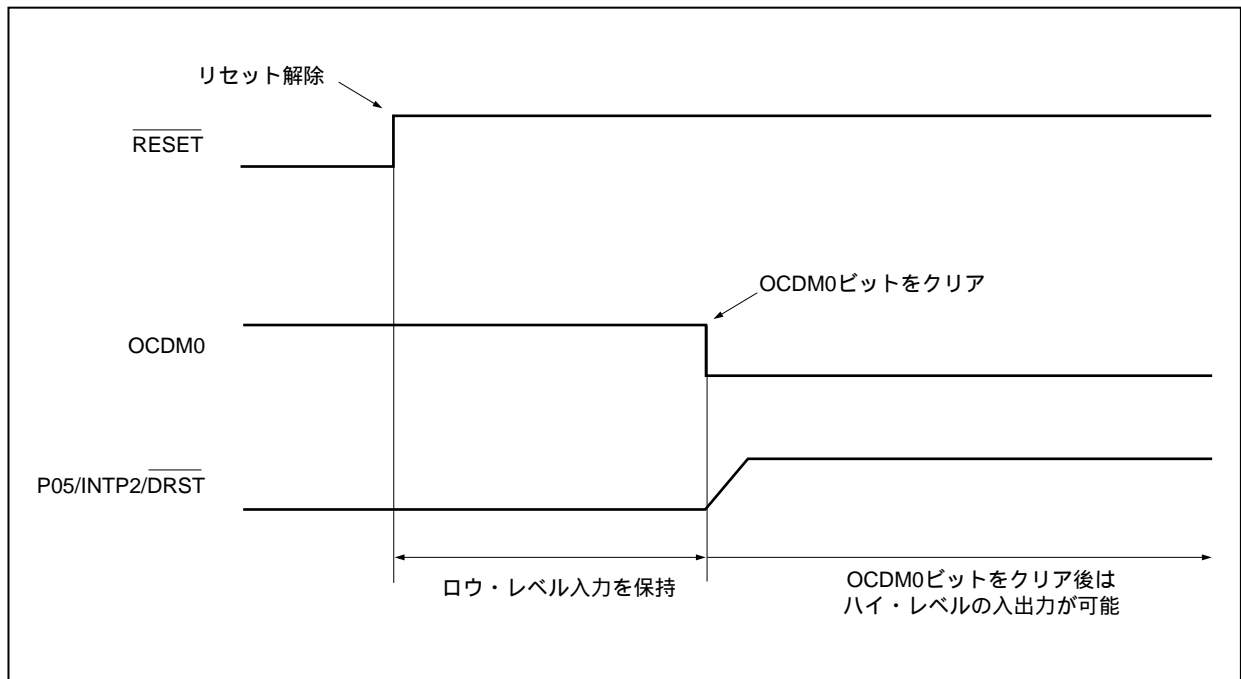
図28 - 1 オンチップ・ディバグ機能未使用時のタイミング
