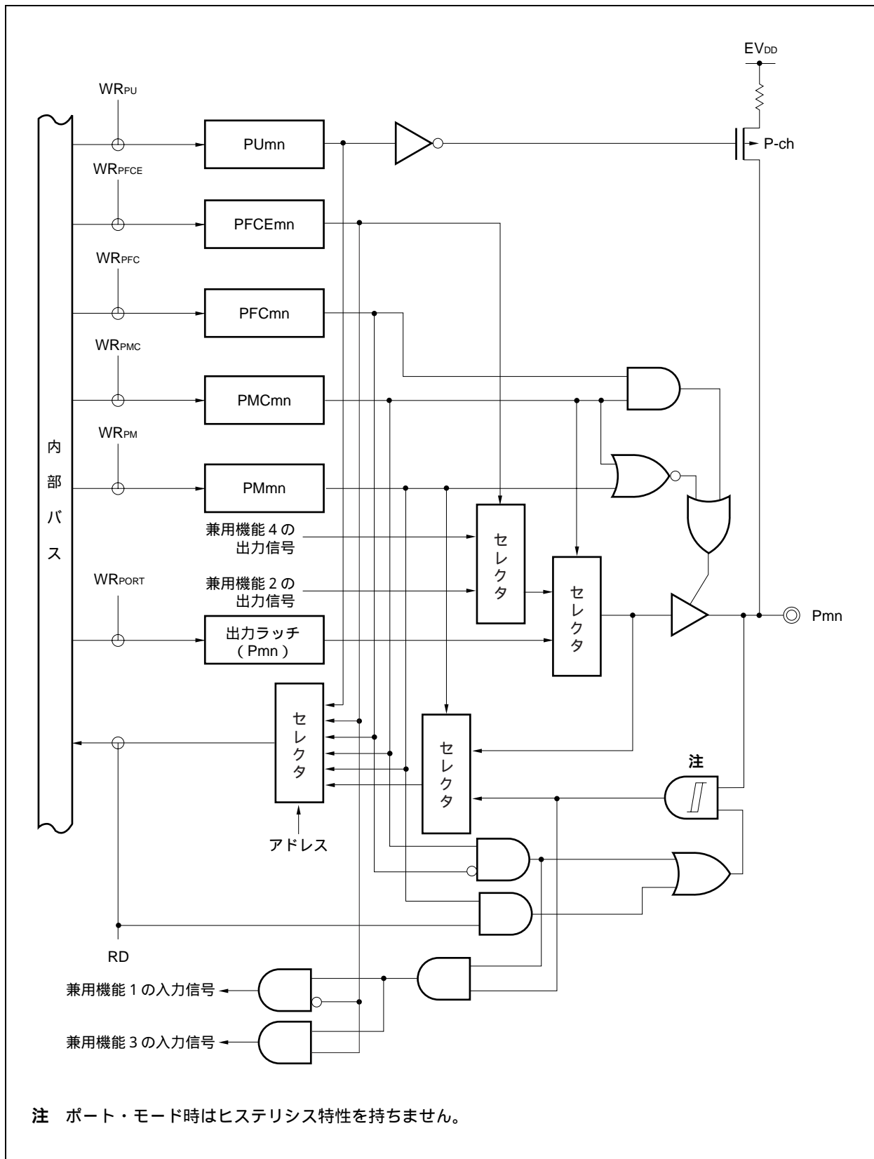
図4 - 26 タイプG-7-1のブロック図
