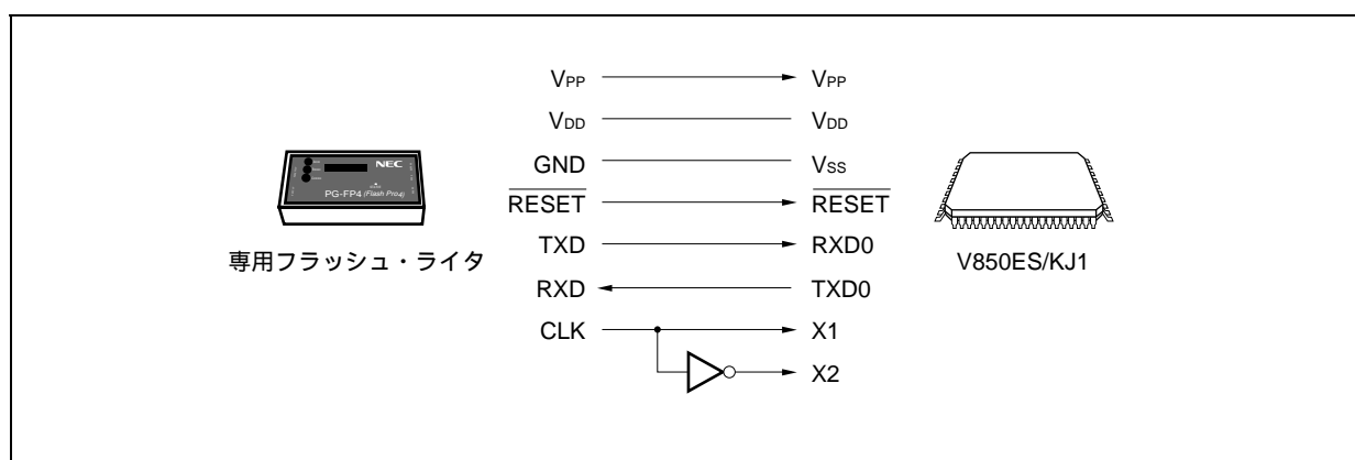
図27-3 専用フラッシュ・ライターとの通信（UART0）
