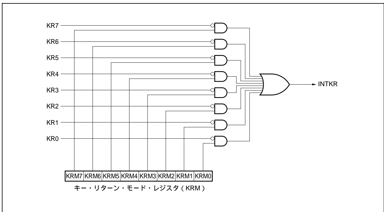
図21 - 1 キー・リターンのブロック図
