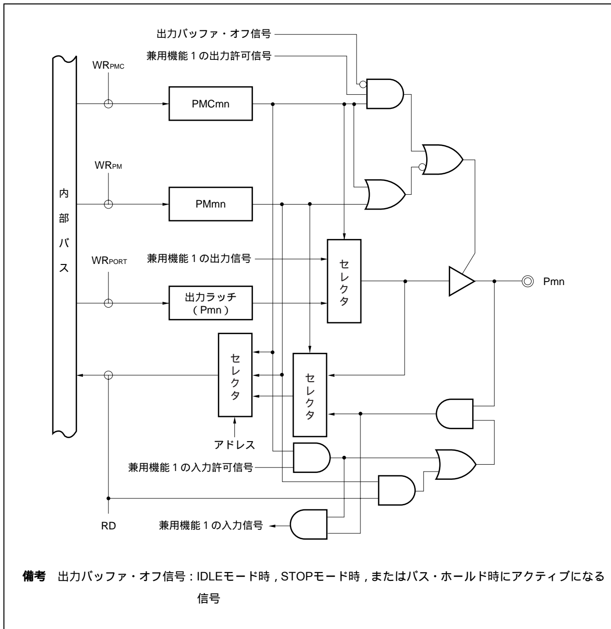
図4 - 8 タイプC-4のブロック図
