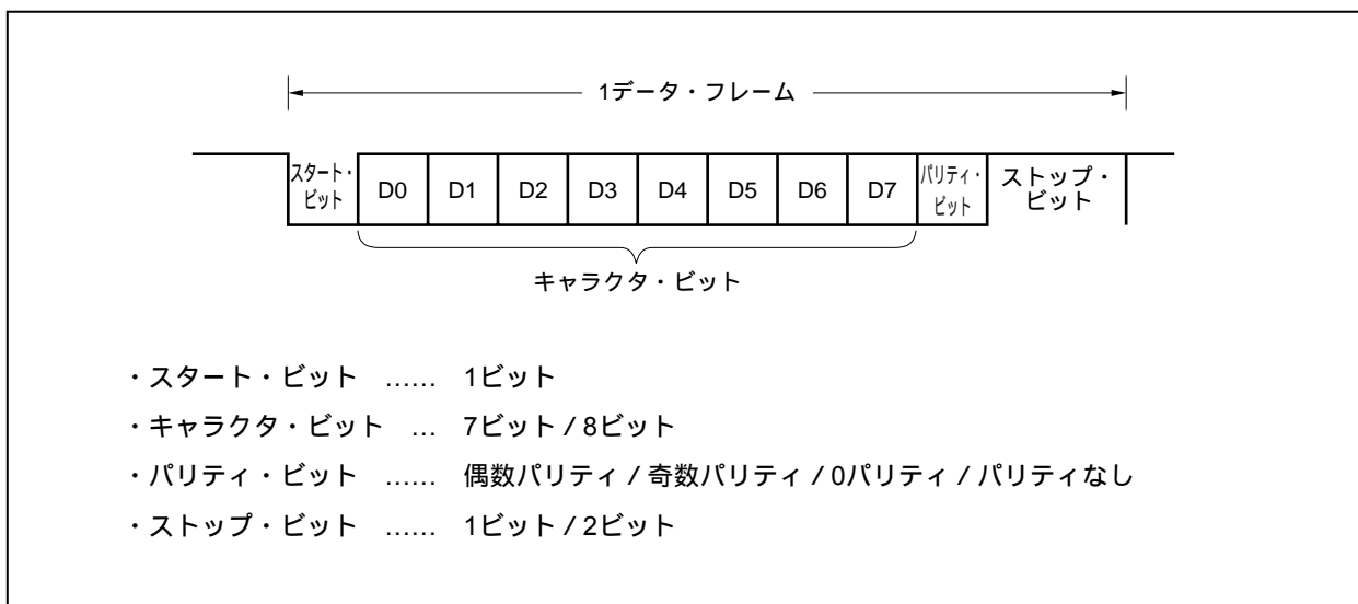
図16-3 UARTnの送受信データのフォーマット
