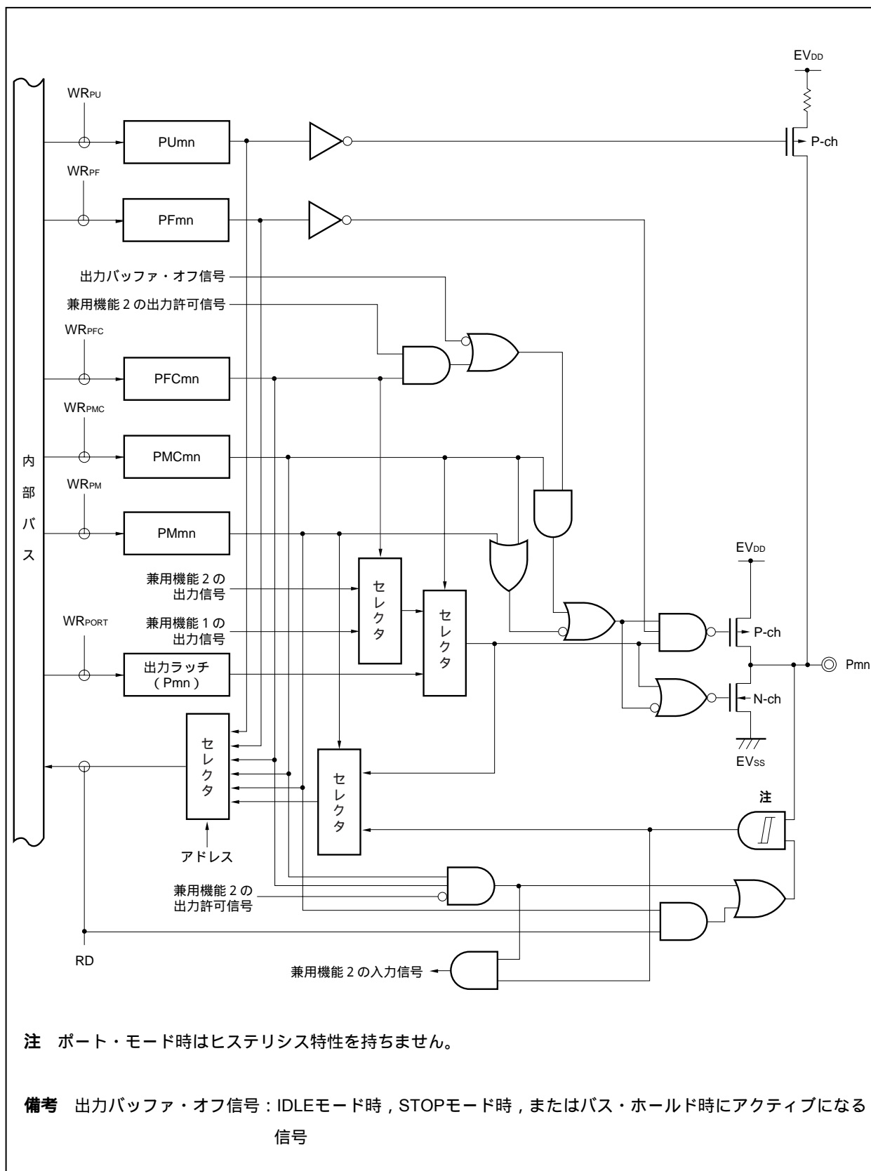
図4-22 タイプG-3のブロック図
