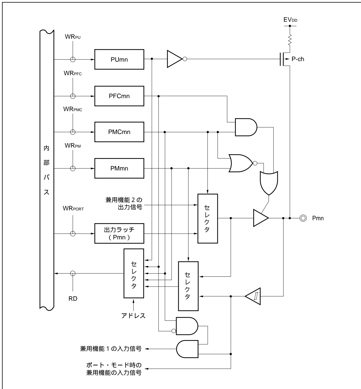
図4 - 16 タイプE-5のブロック図
