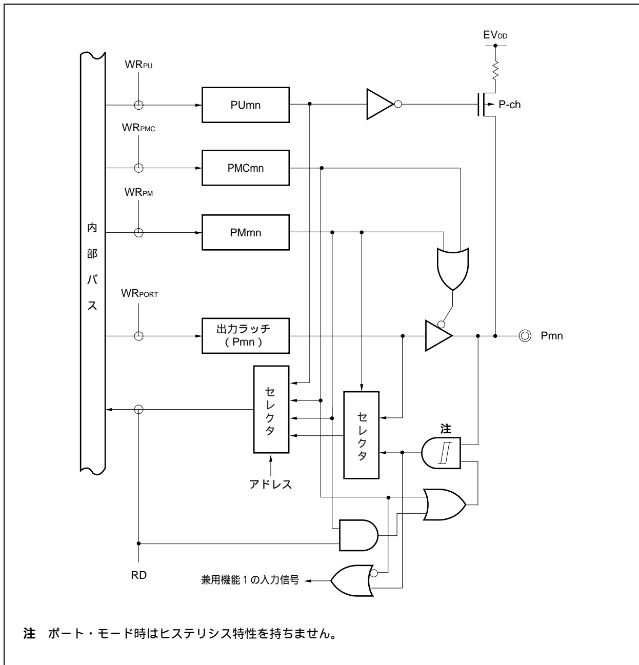
図4-9 タイプD-1-1のブロック図
