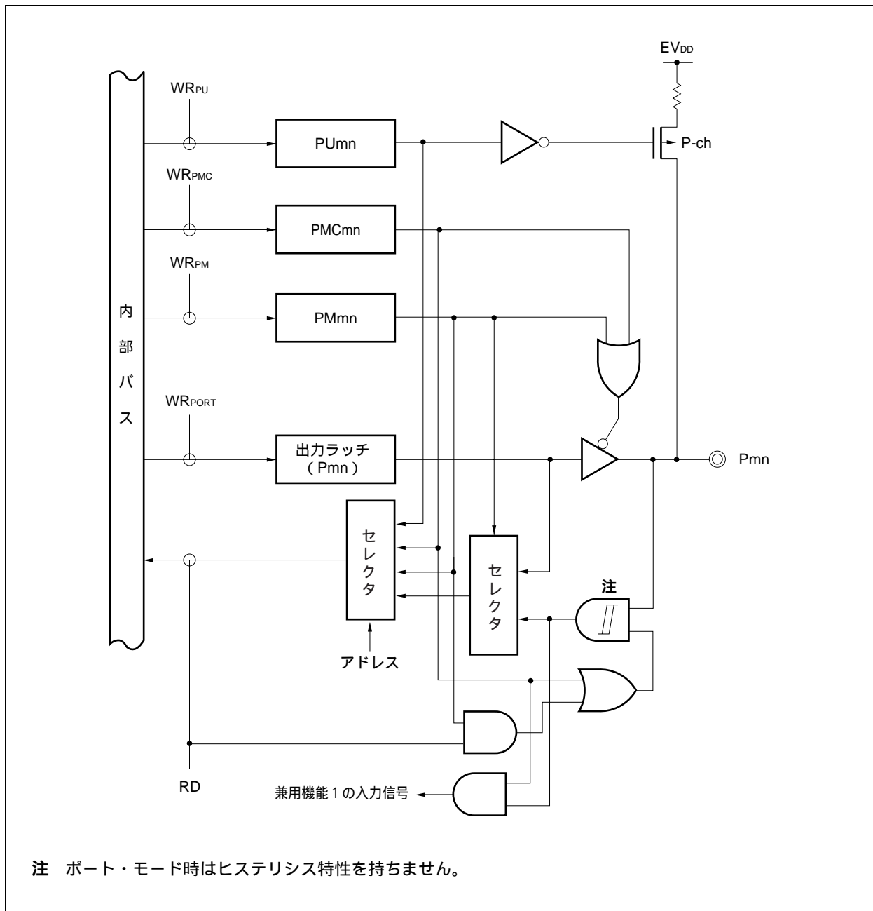
図4 - 10 タイプD-1-2のブロック図
