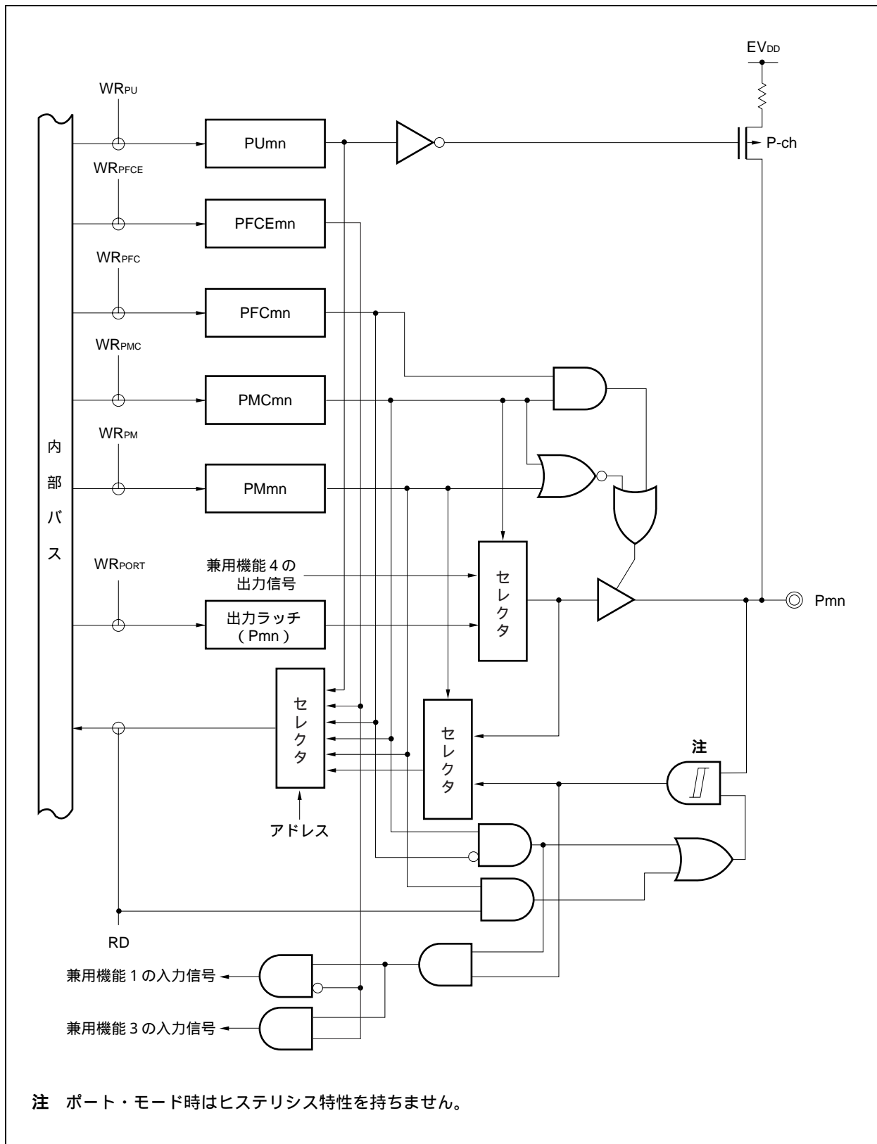
図4-27 タイプG-7-2のブロック図
