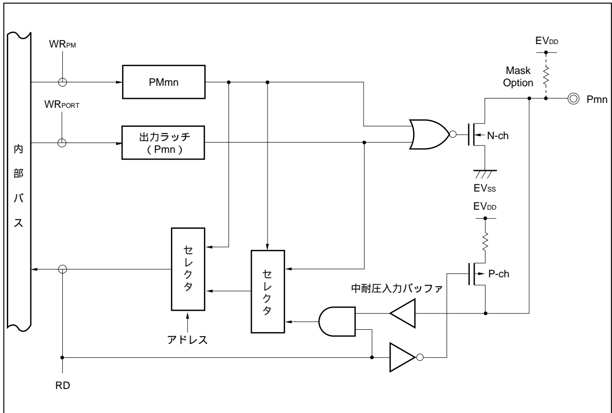
図4 - 30 タイプJのブロック図
