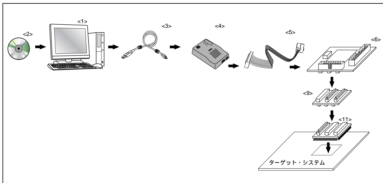
図A - 5 QB-V850ESKX1-DAを使用したシステム構成（オプション製品を使用しない場合）
