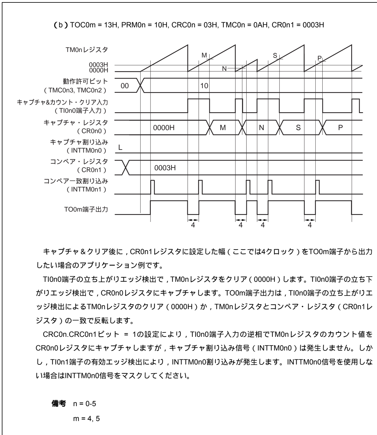
図8 - 18 TI0n0端子の有効エッジ入力によるクリア&スタート・モードのタイミング例 (CR0n0レジスタ：キャプチャ・レジスタ/CR0n1レジスタ：コンペア・レジスタ) (2/2)
