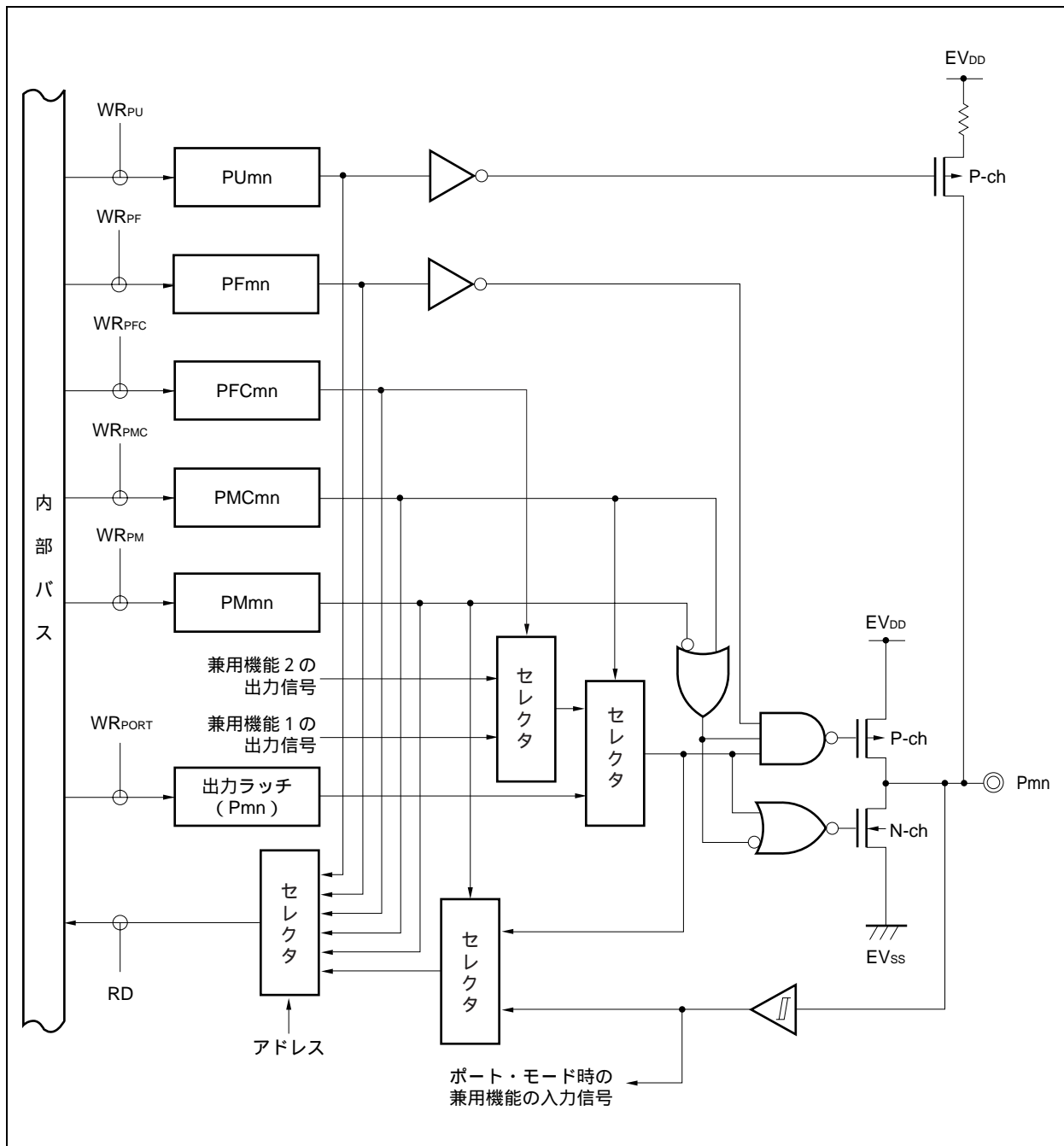
図4 - 20 タイプG-1のブロック図
