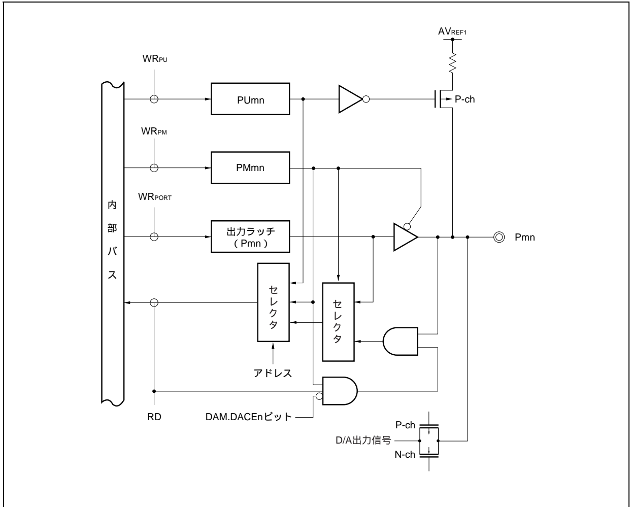
図4 - 3 タイプA-2のブロック図
