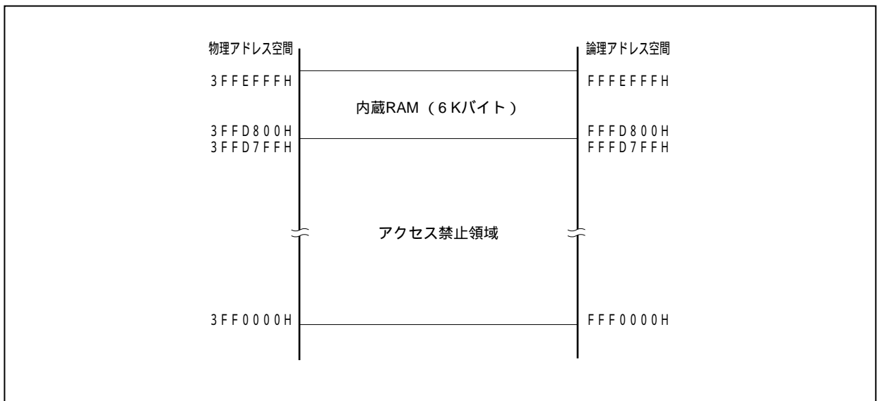
図3 - 8 内蔵RAM (6 Kバイト)
