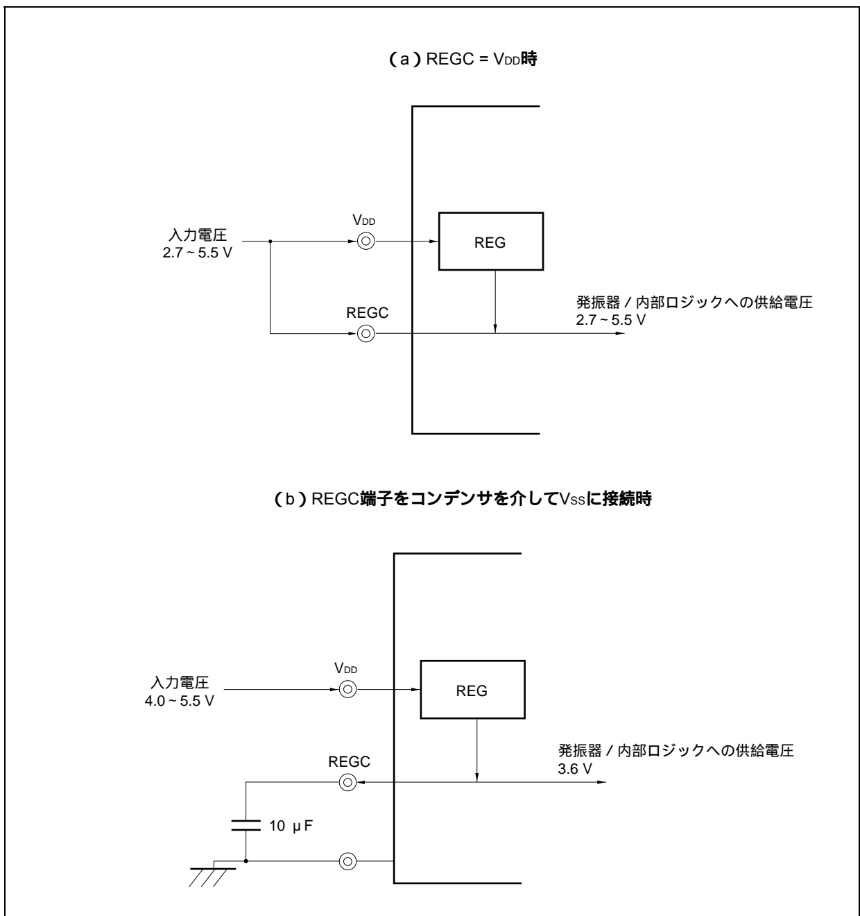
図24 - 2 REGC 端子の接続
