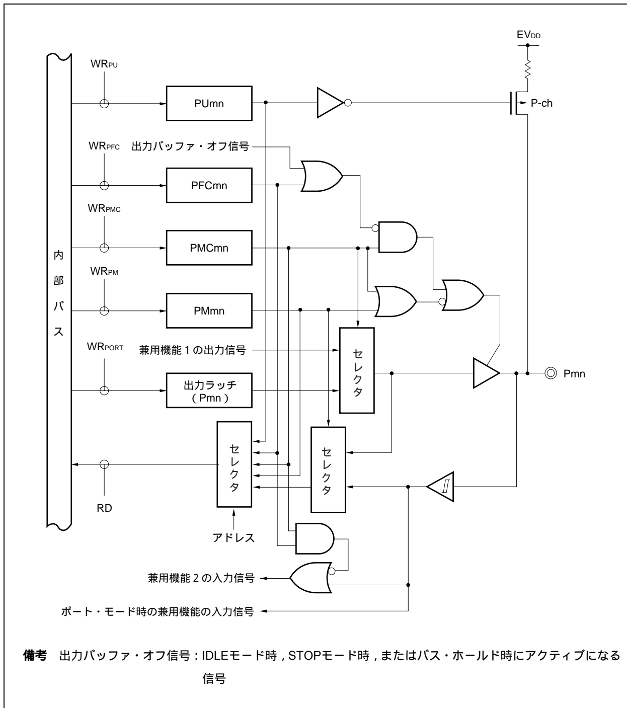
図4 - 12 タイプE-1のブロック図
