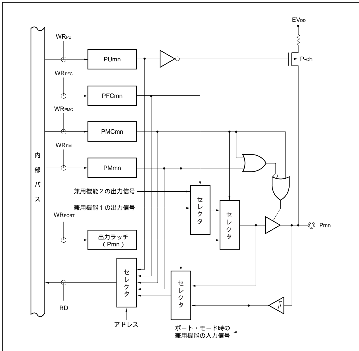
図4 - 15 タイプE-4のブロック図
