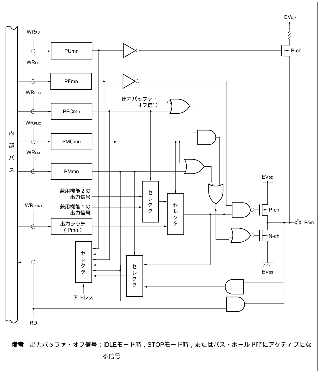
図4-23 タイプG-4のブロック図
