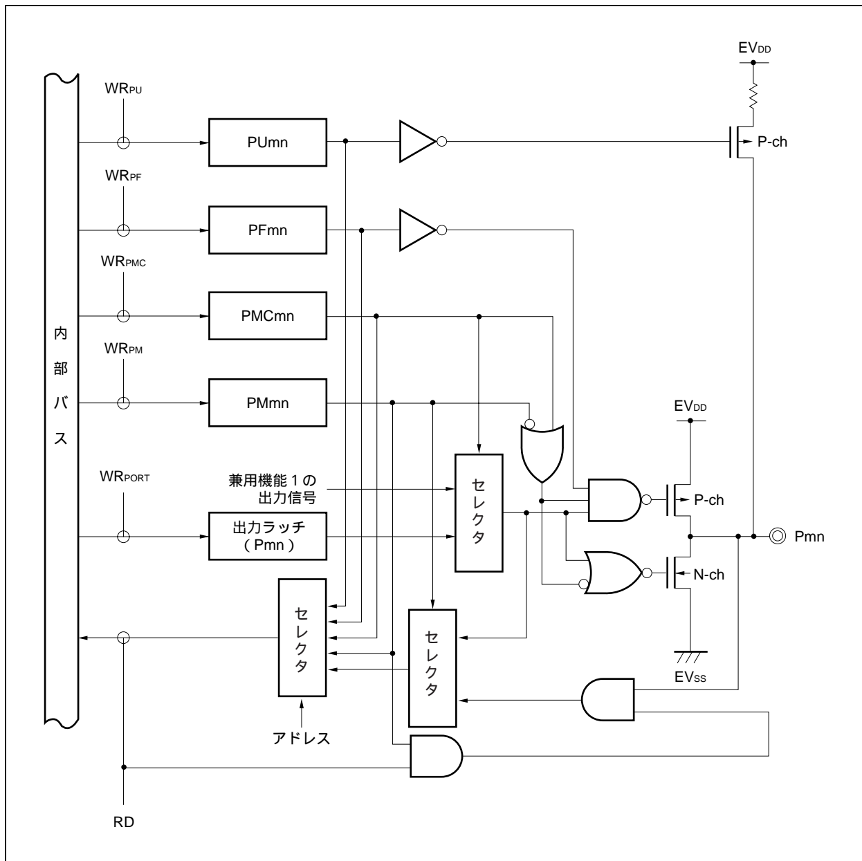
図4 - 18 タイプF-1のブロック図
