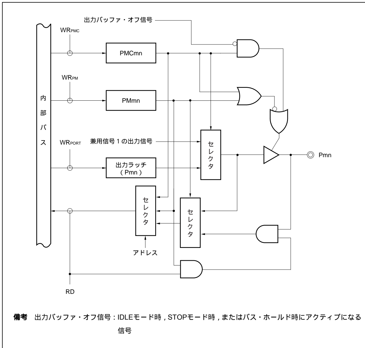
図4-7 タイプC-3のブロック図
