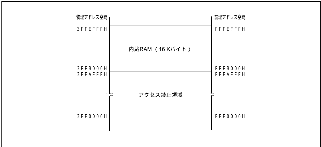
図3 - 7 内蔵RAM (16 Kバイト)
