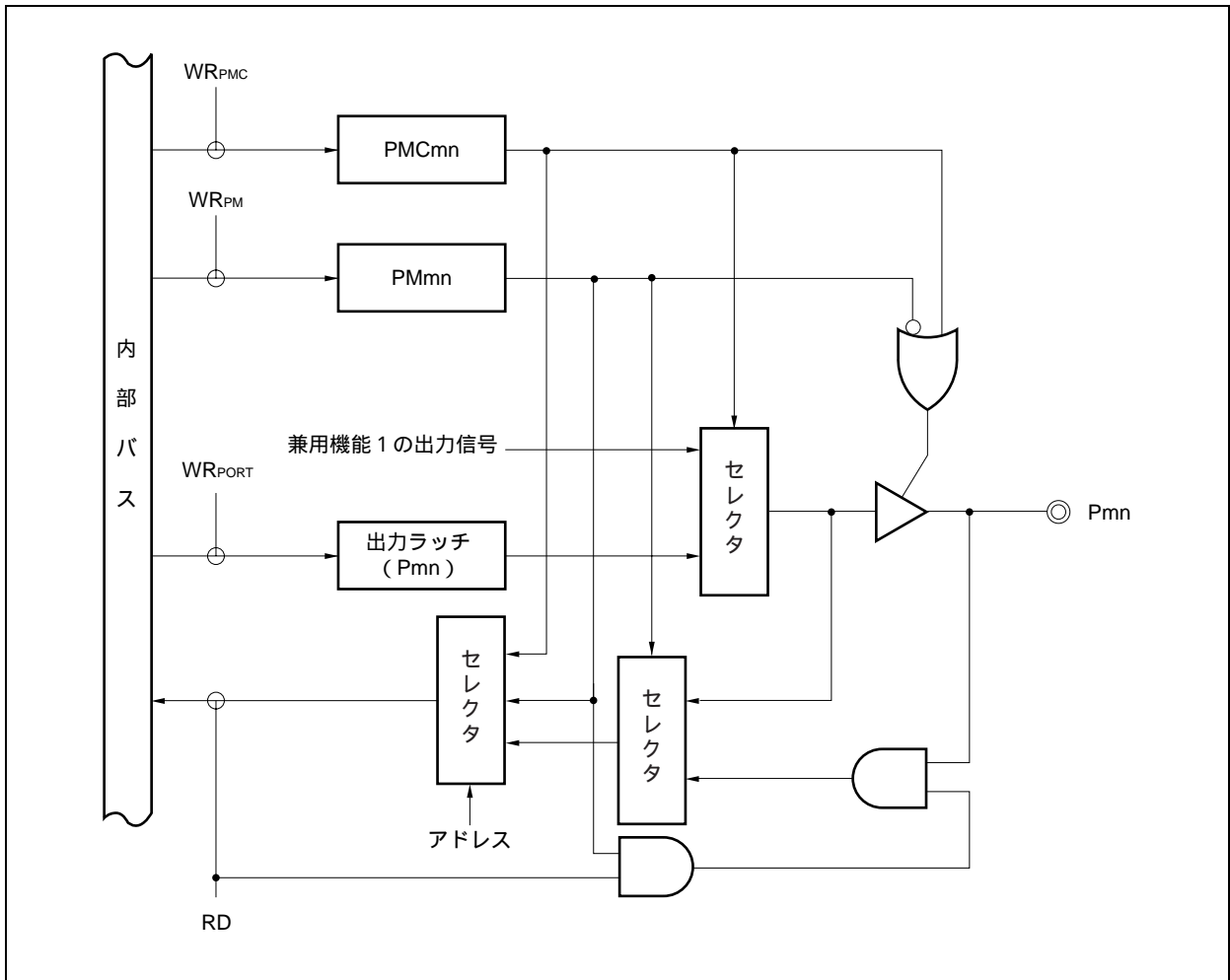
図4 - 6 タイプC-2のブロック図
