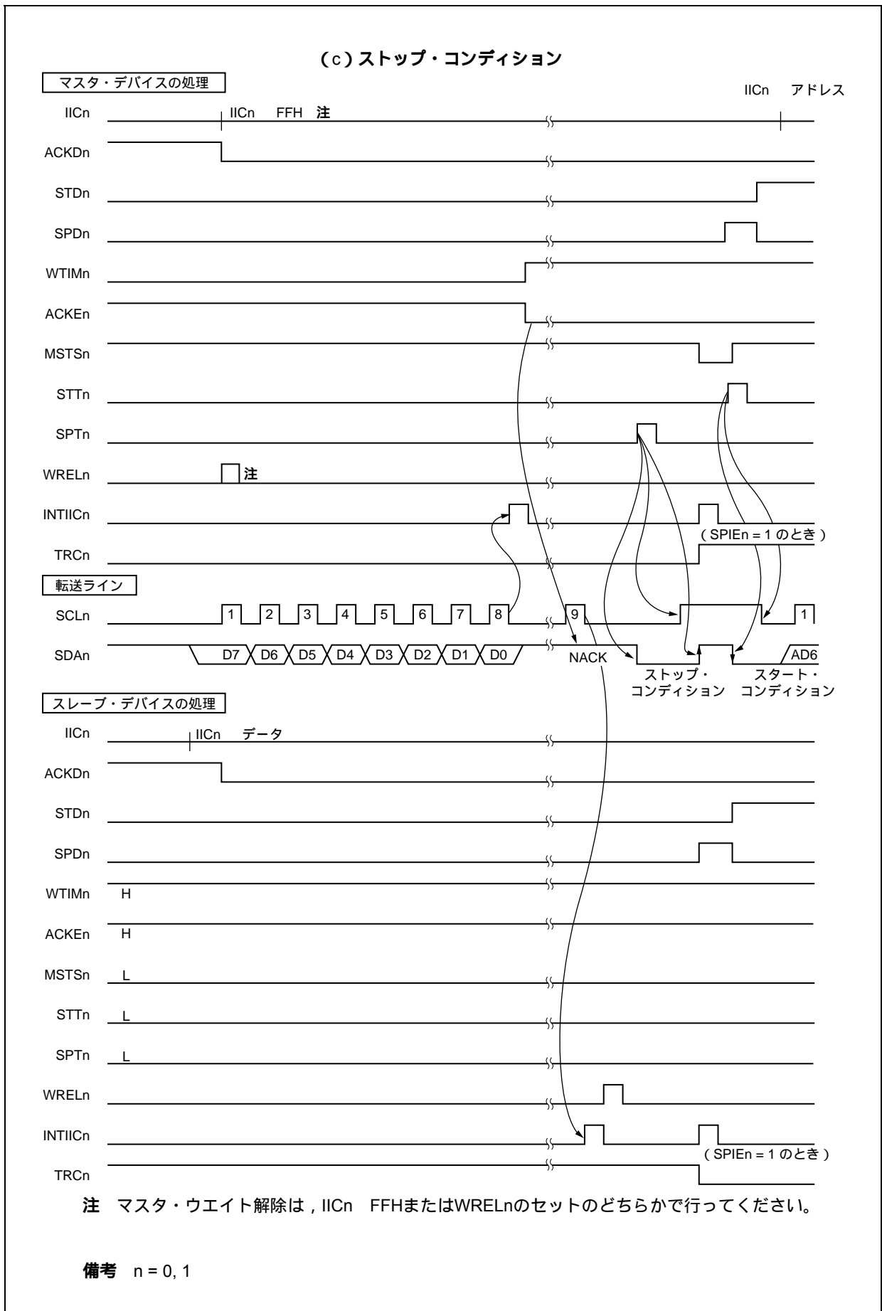
★ 図19-22 スレーブ マスタ通信例 (マスタ:8 9クロック, スレーブ:9クロックでウエイト選択時) (3/3)
