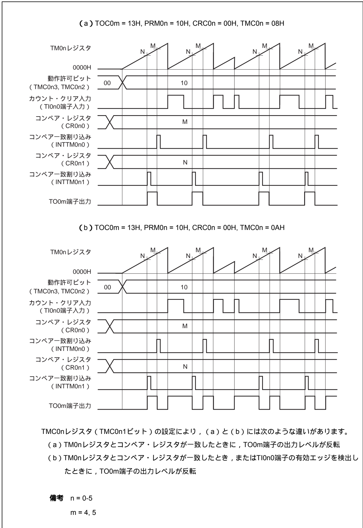
図8 - 14 TI0n0端子の有効エッジ入力によるクリア&スタート・モードのタイミング例 (CR0n0レジスタ：コンペア・レジスタ / CR0n1レジスタ：コンペア・レジスタ)
