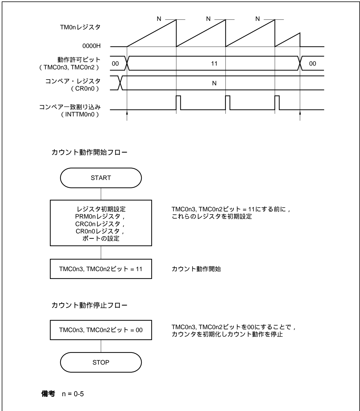
図8-5 インターバル・タイマ機能時のソフトウェア処理機能
