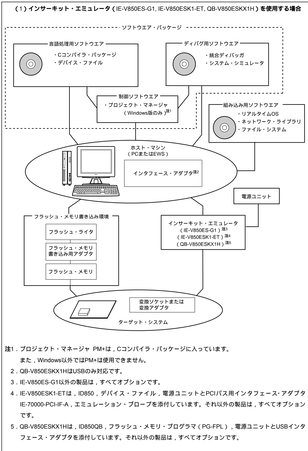
図A - 1 開発ツール構成 (1/2)
