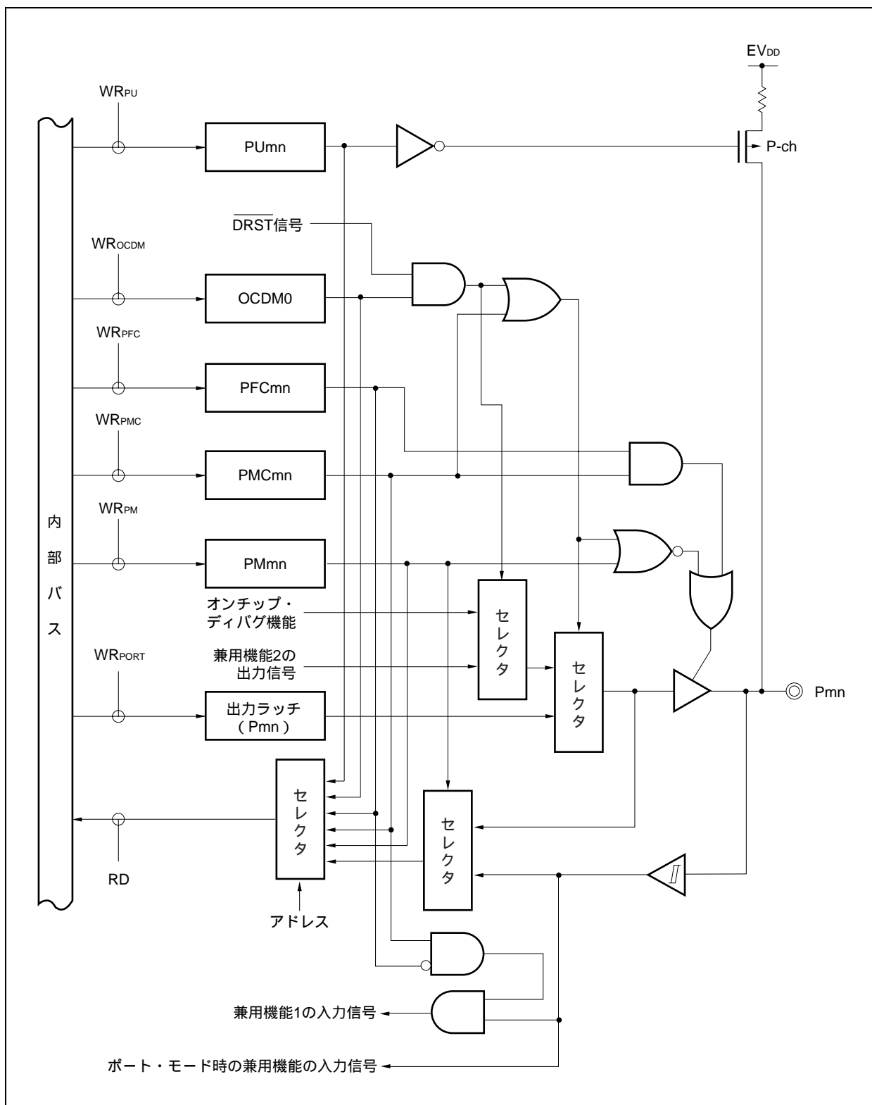
図4 - 35 タイプO-4のブロック図
