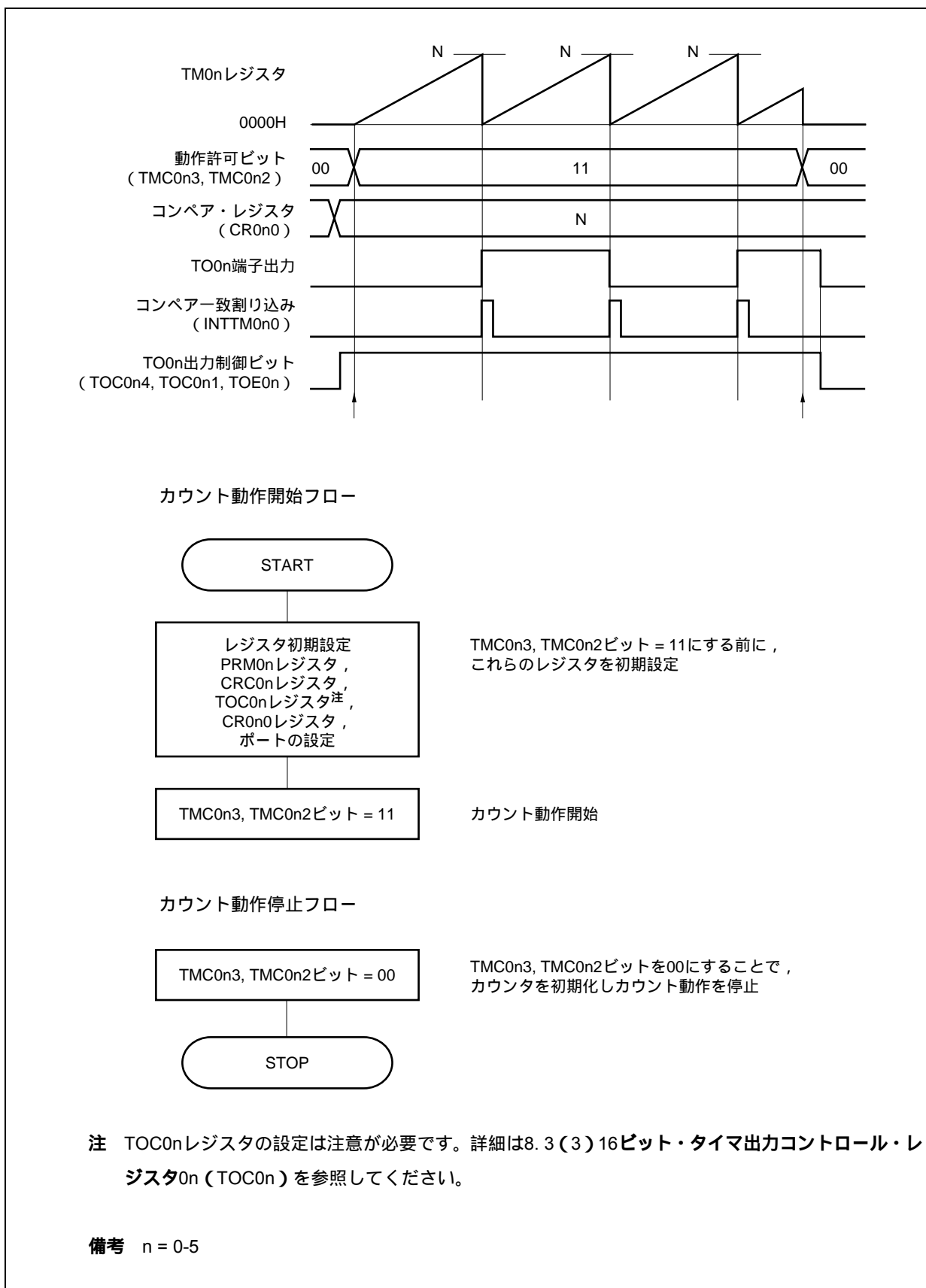
図8 - 12 外部イベント・カウンタ・モード動作時のソフトウェア処理例
