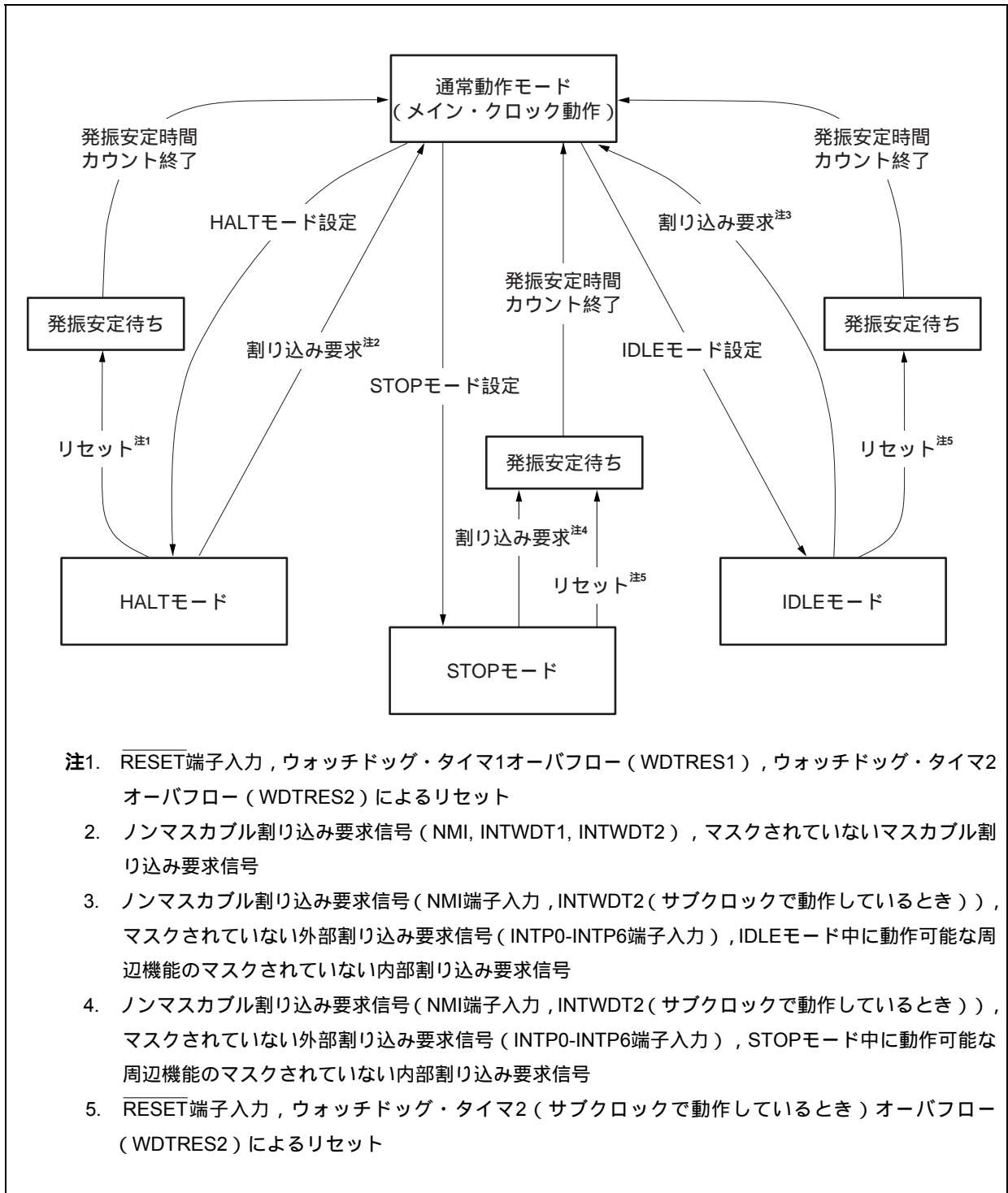
図22 - 1 状態遷移図 (1/2)
