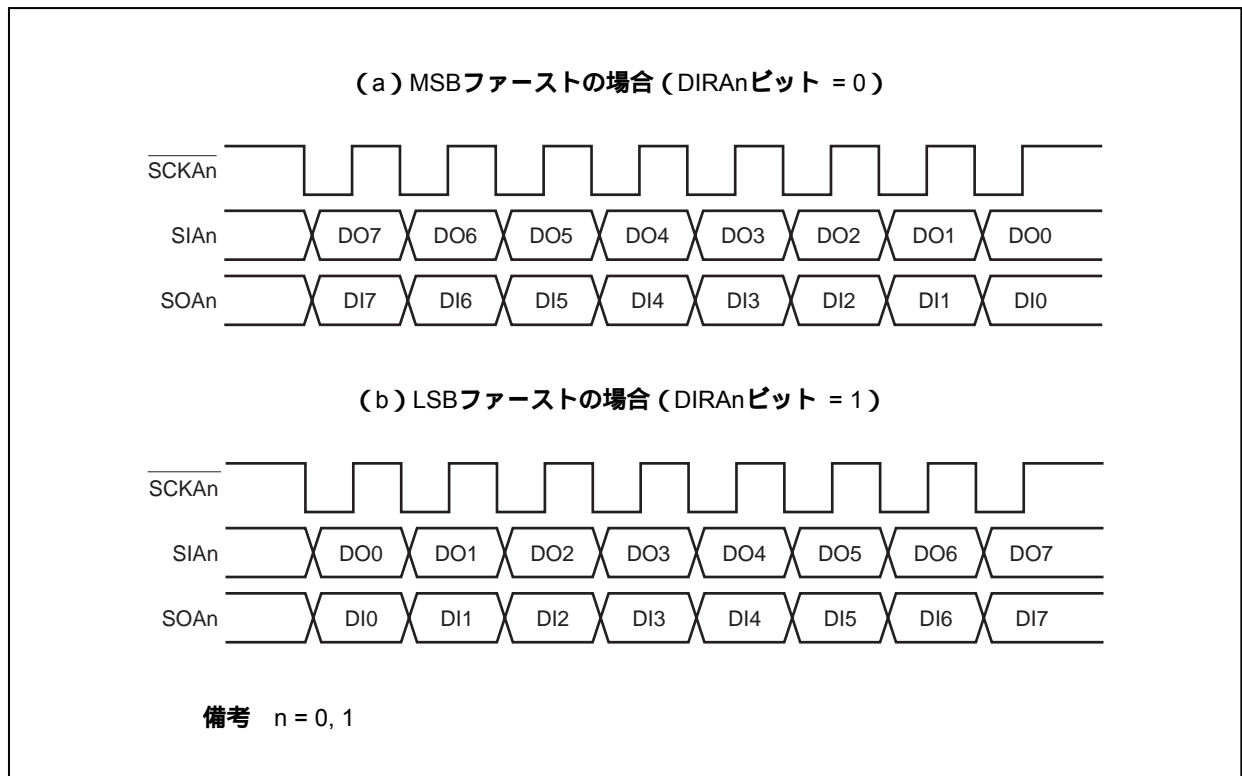
図18 - 14 CSIA n の送受信データのフォーマット
