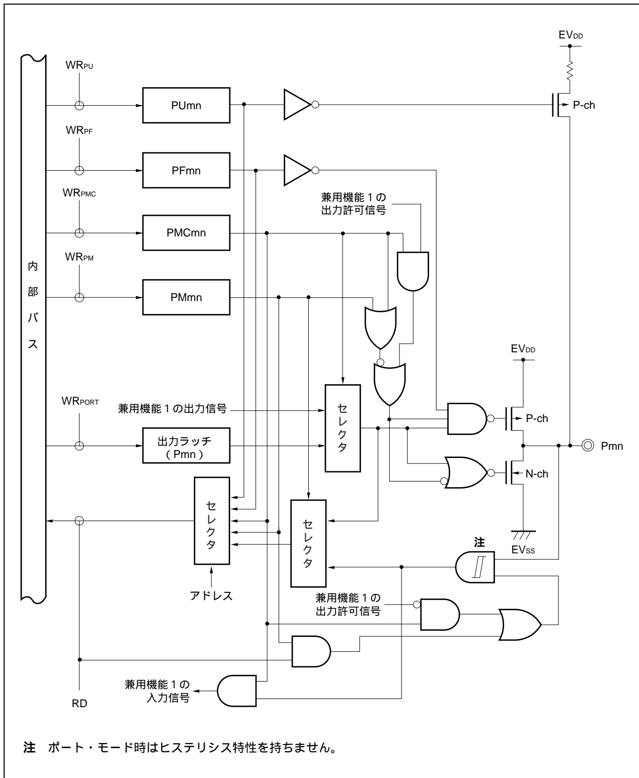
図4 - 19 タイプF-2のブロック図
