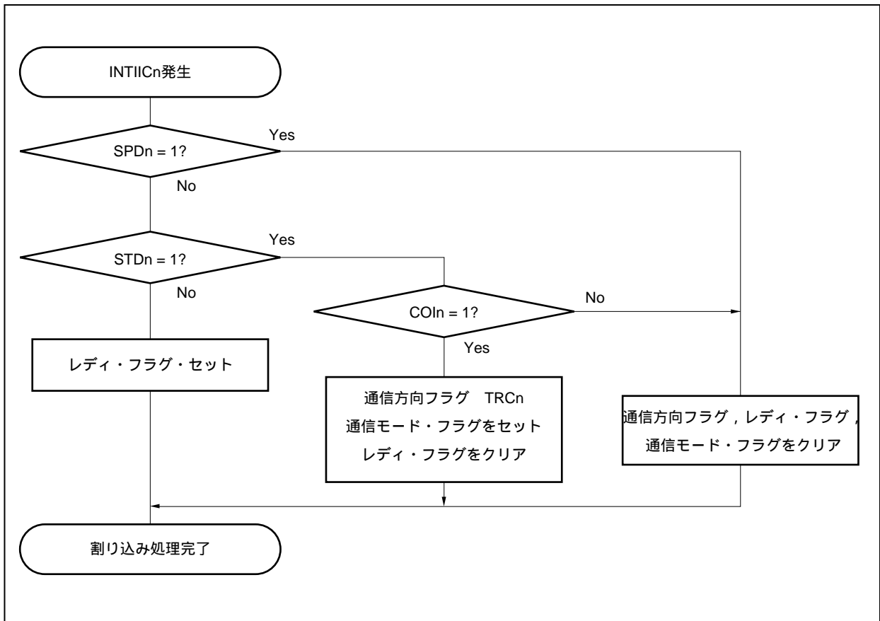
図19-20 スレーブ動作手順(2)
