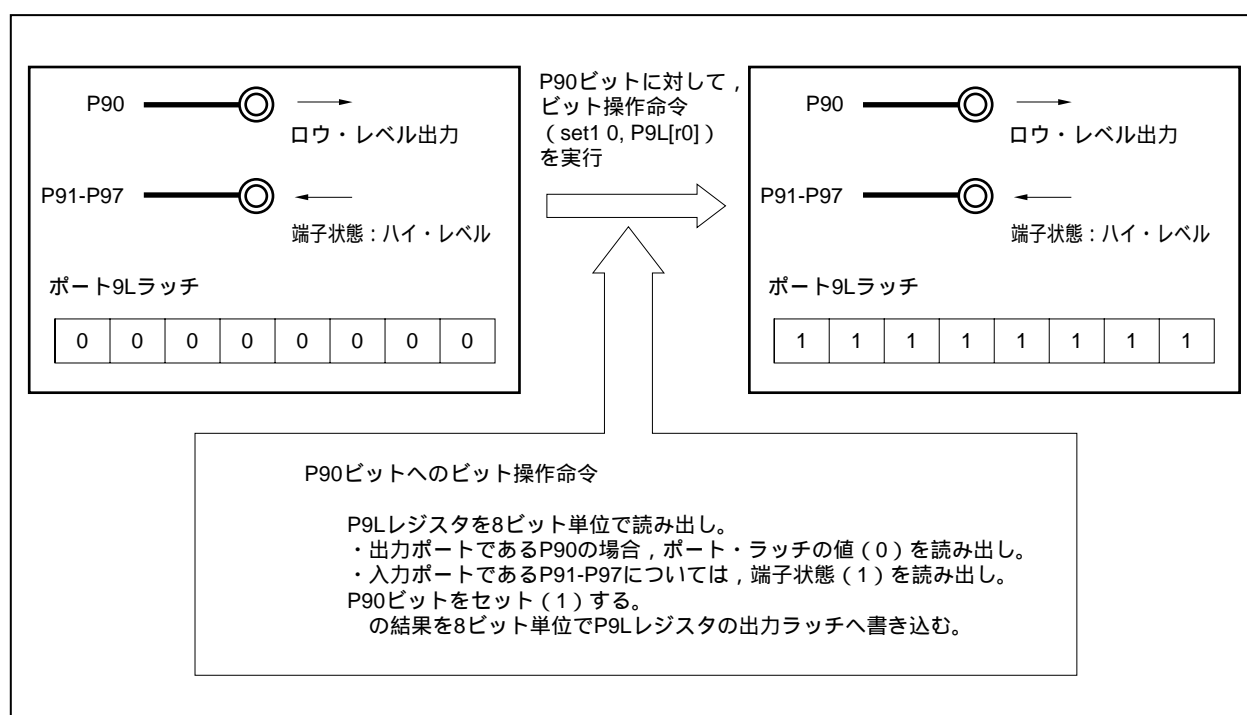
図4 - 37 ビット操作命令 (P90の場合)
