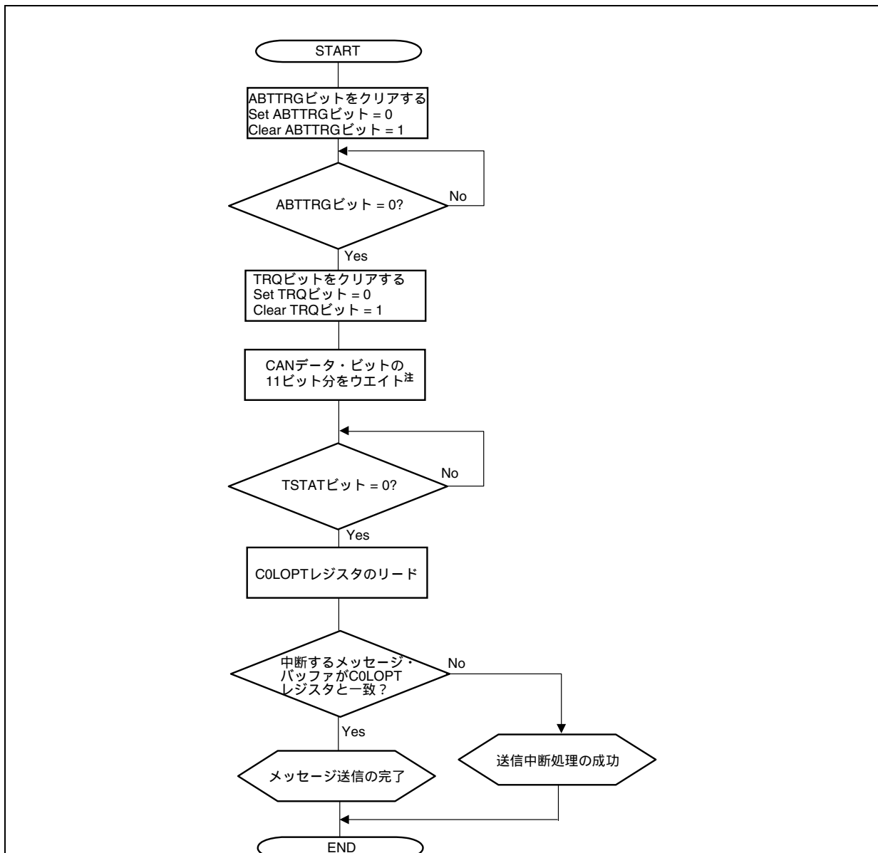
図19 - 47 ABT送信以外の送信中断処理 (ABT付き通常動作モード)
