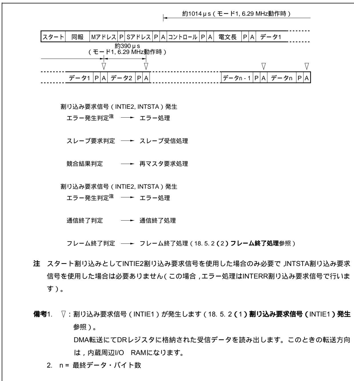
図18 - 27 マスタ受信
