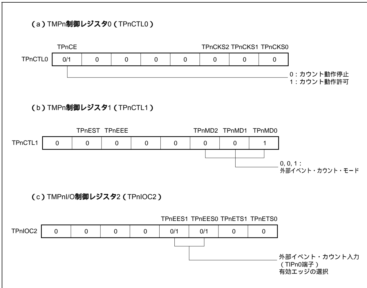
図7 - 15 外部イベント・カウンタ・モード動作時のレジスタ設定内容(1/2)
