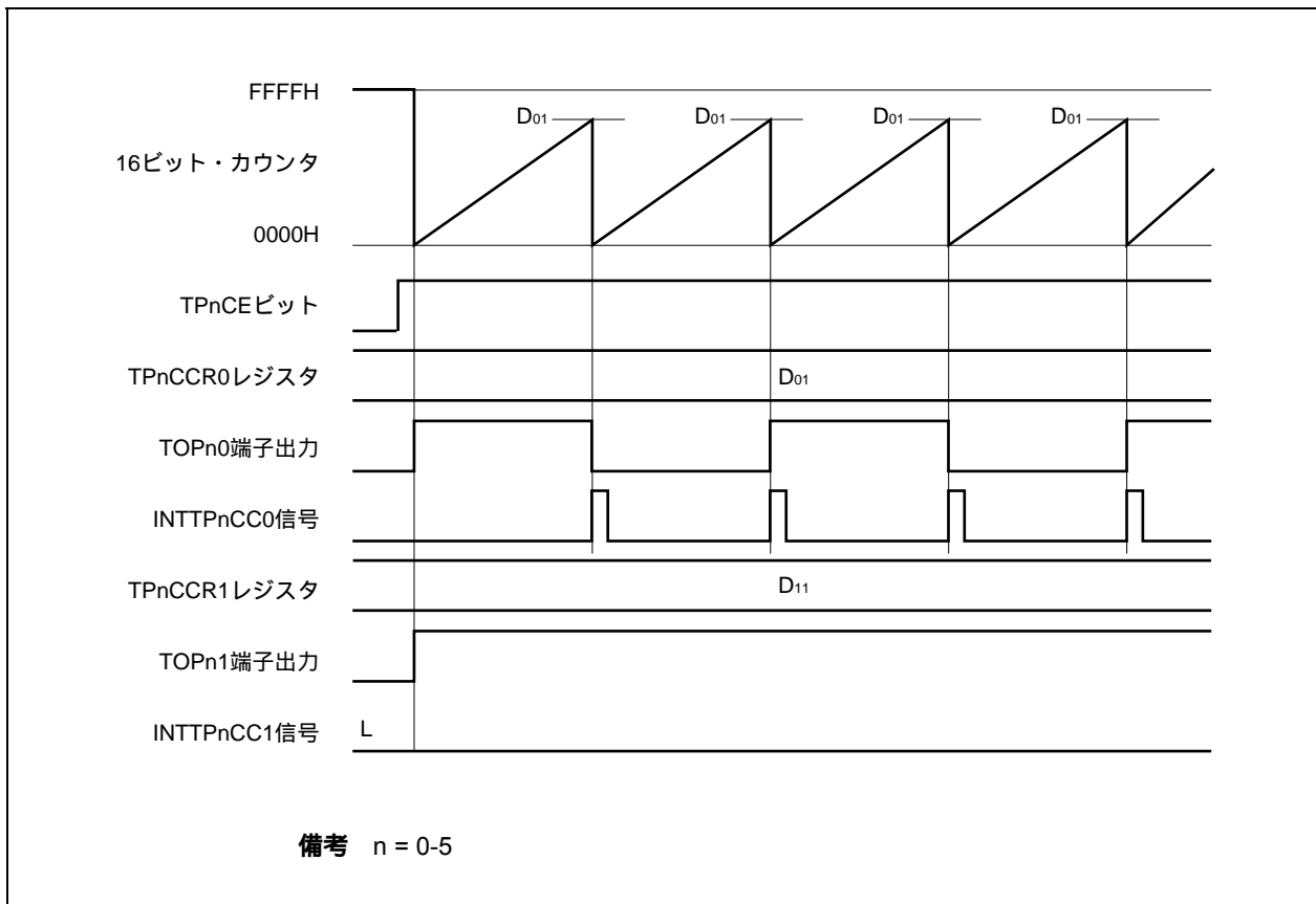
図7 - 12 D 01 < D 11 の場合のタイミング図
