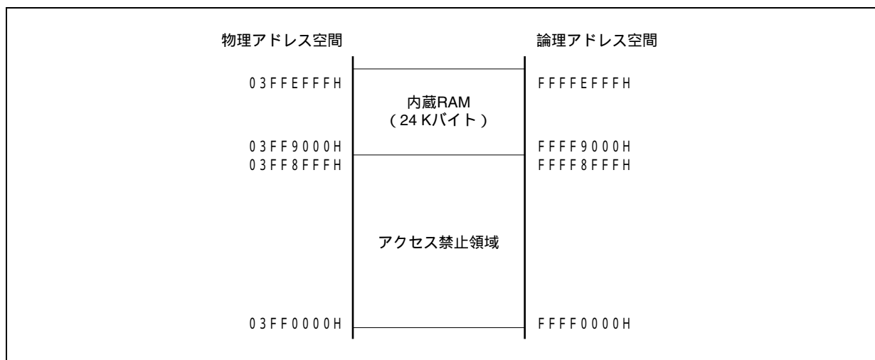
図3 - 8 内蔵RAM領域 (24 Kバイト)
