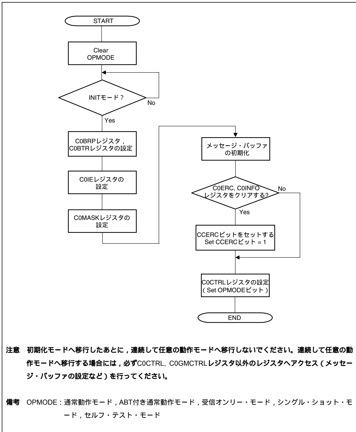
図19 - 37 再初期化
