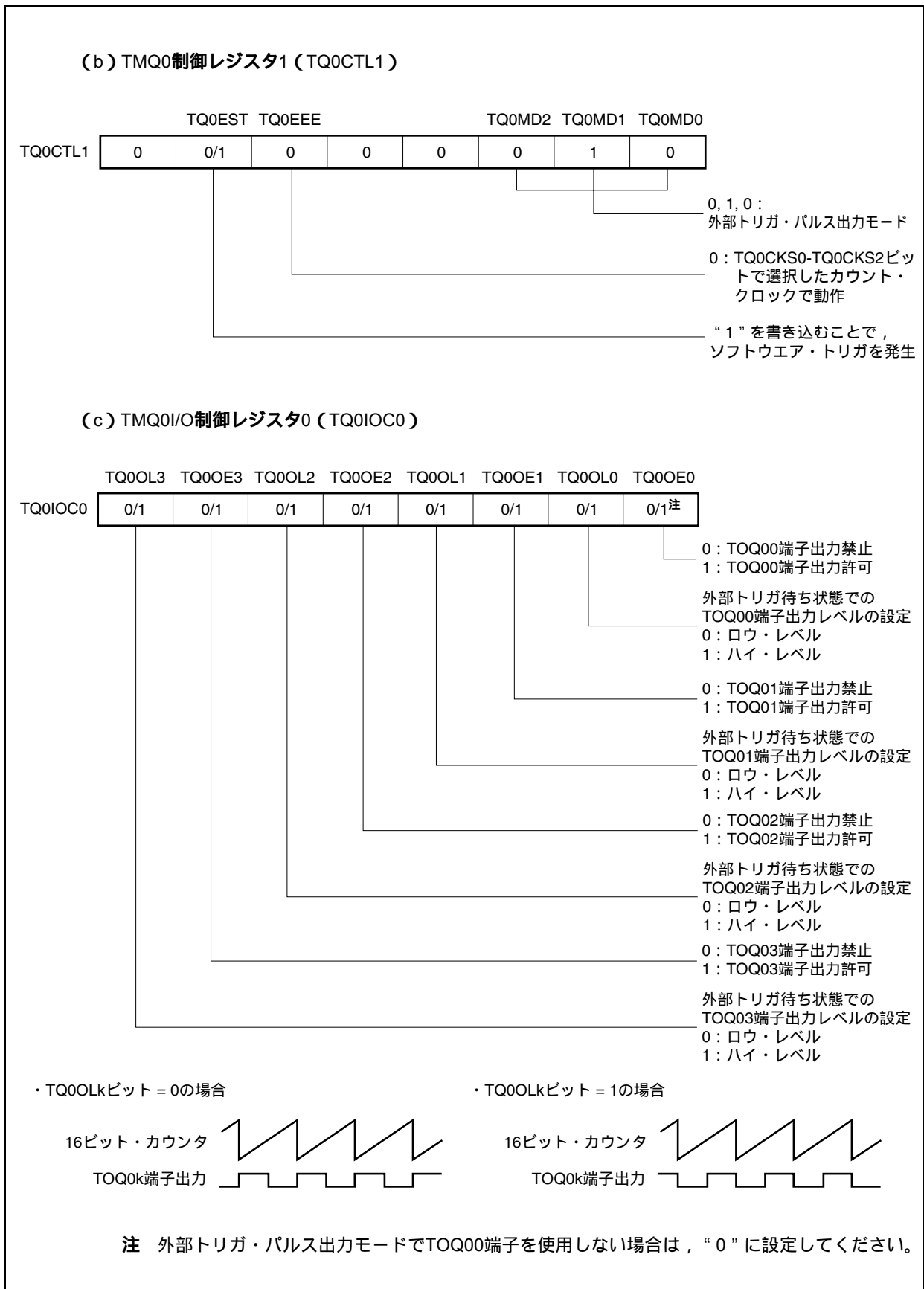
図8 - 22 外部トリガ・パルス出力モード動作時のレジスタ設定内容 (2/3)
