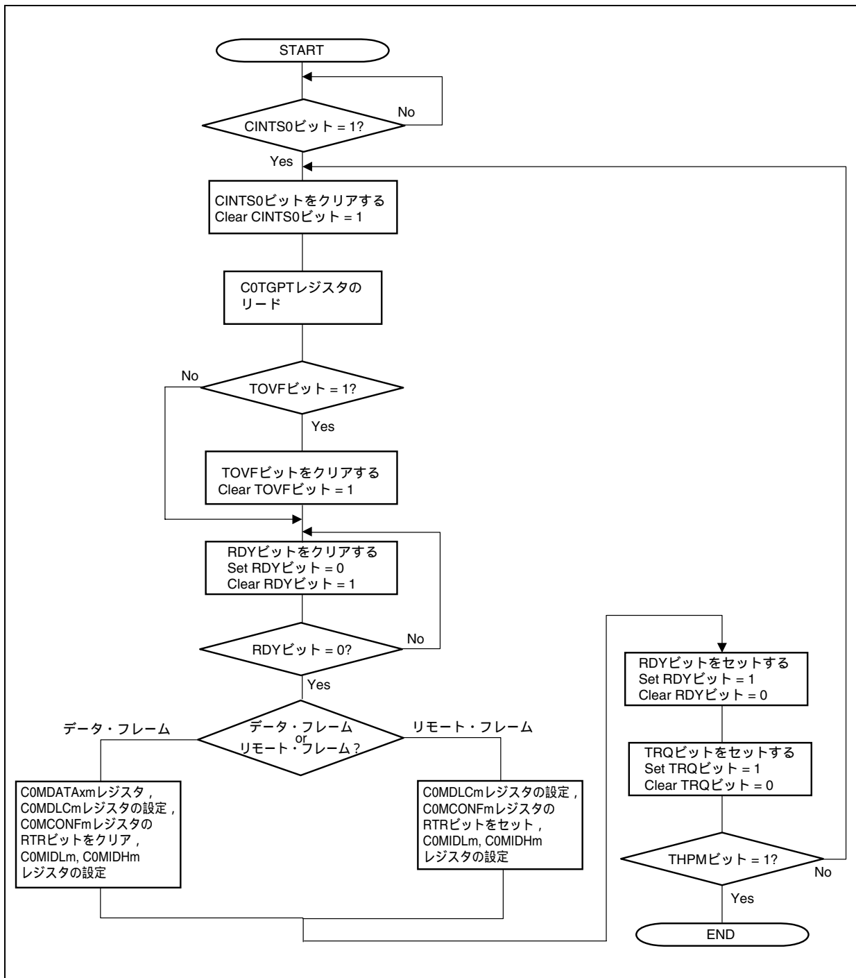
図19 - 45 ソフトウェア・ポーリングによる送信処理
