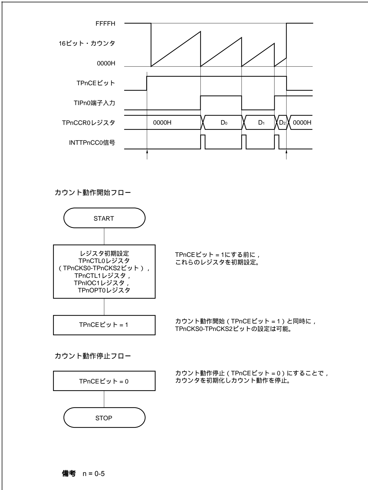
図7 - 41 パルス幅測定モード使用時のソフトウェア処理フロー
