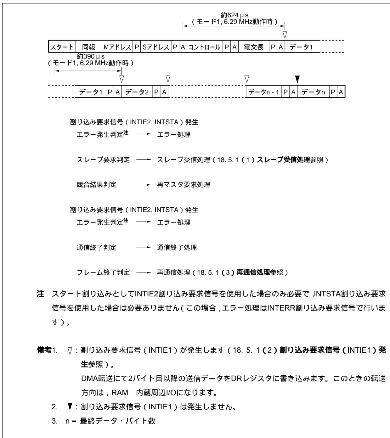
図18 - 26 マスタ送信
