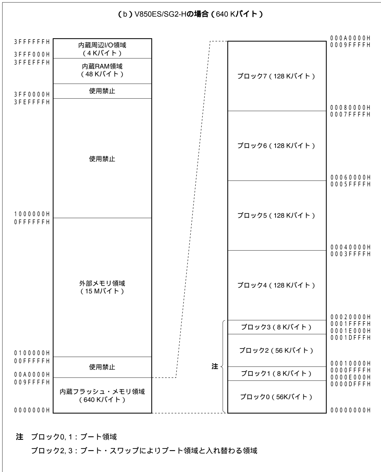
図30 - 1 フラッシュ・メモリ・マッピング (2/2)
