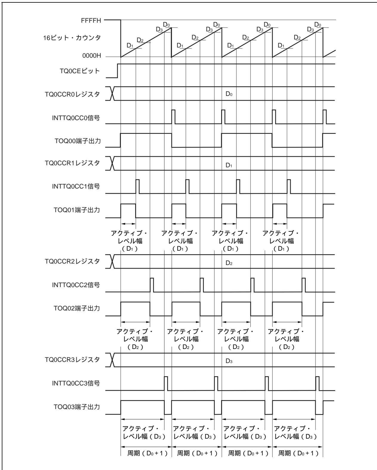
図8 - 29 PWM出力モードの基本タイミング
