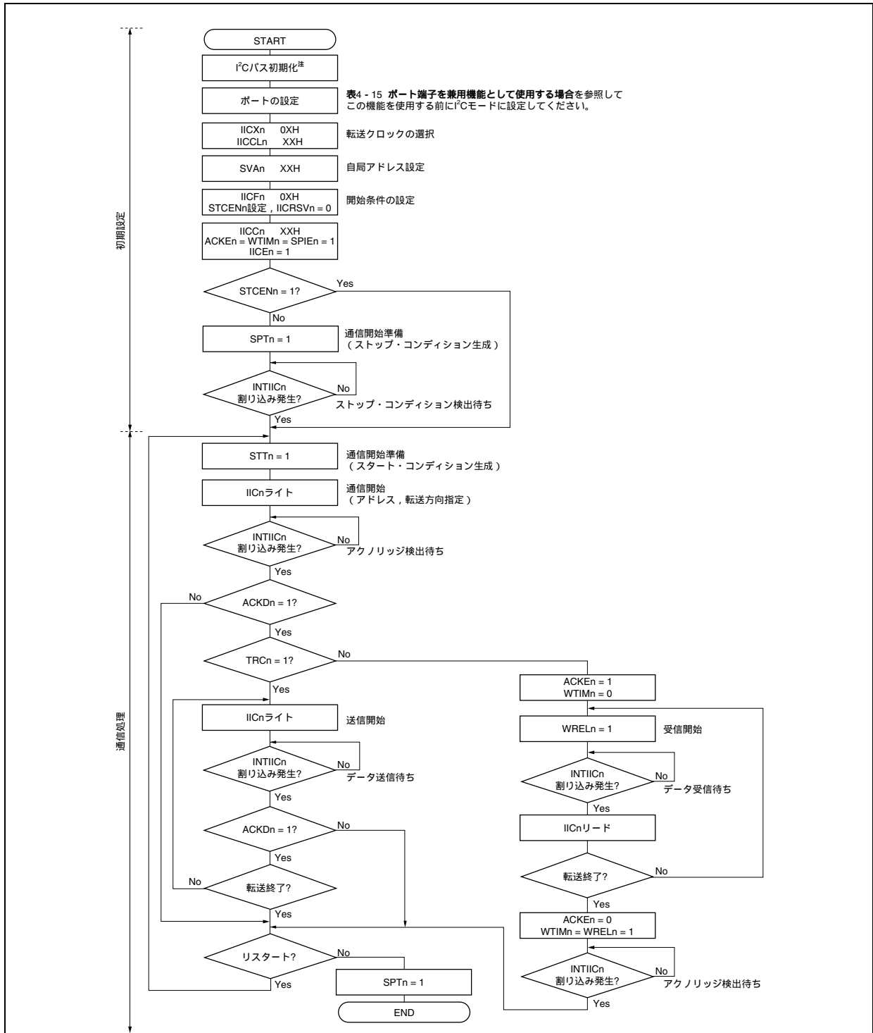
図17-18 シングルマスタ・システムでのマスタ動作
