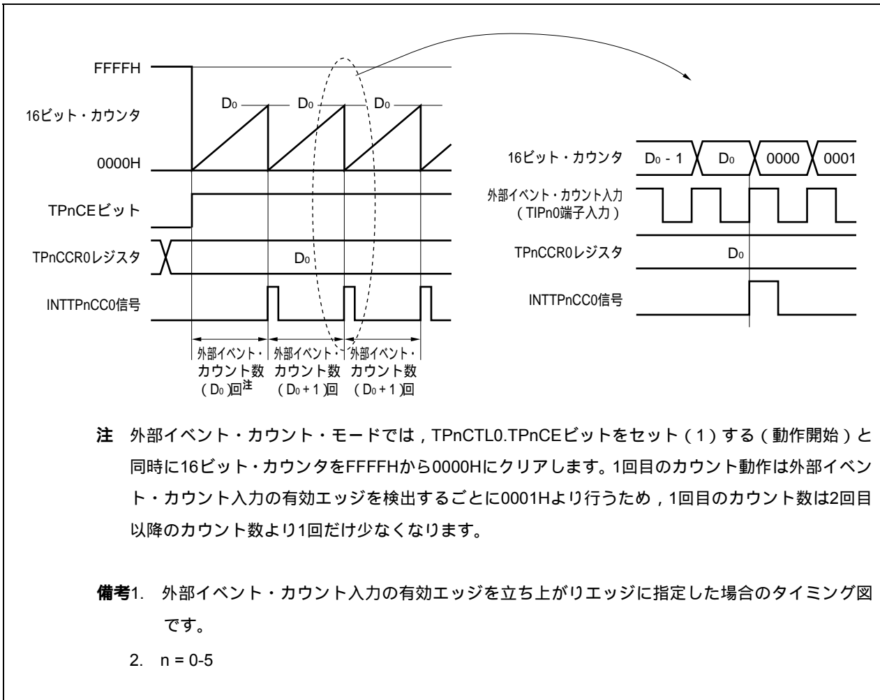
図7-14 外部イベント・カウント・モードの基本タイミング
