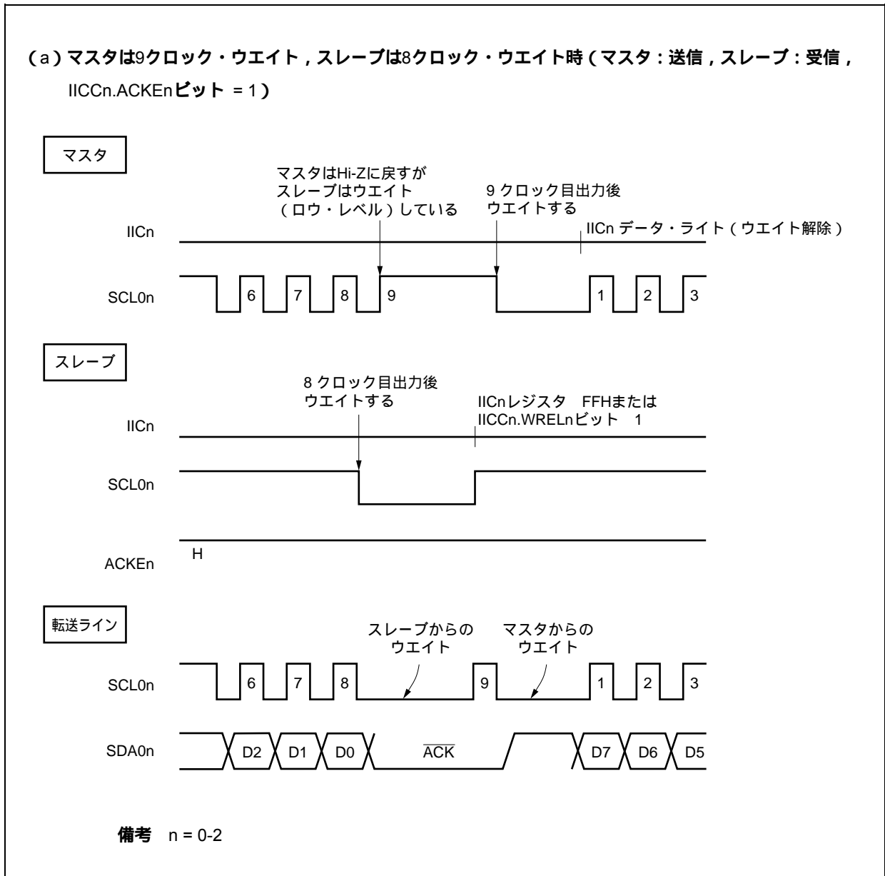
図17 - 13 ウェイト (1/2)
