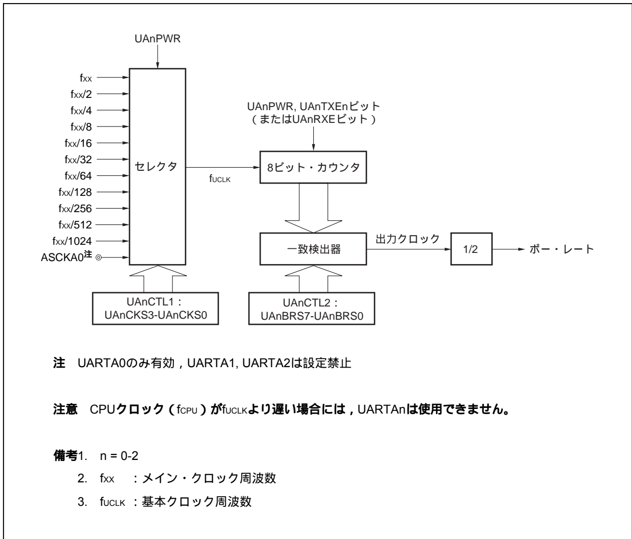
図15 - 16 ポー・レート・ジェネレータの構成
