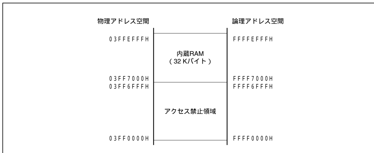
図3 - 9 内蔵RAM領域 (32 Kバイト)
