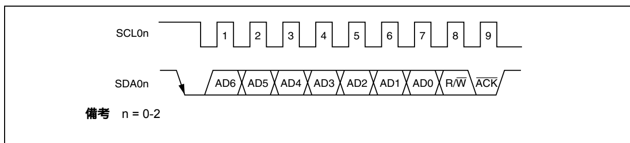
図17-11 アクノリッジ ( \overline{\text{ACK}} )
