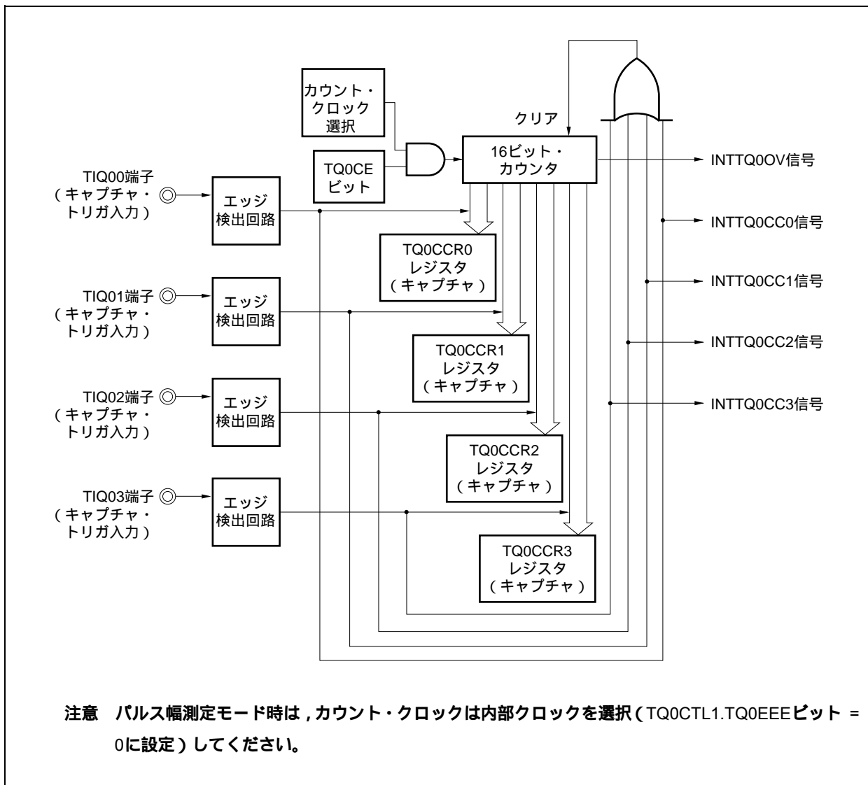
図8-38 パルス幅測定モードの構成図
