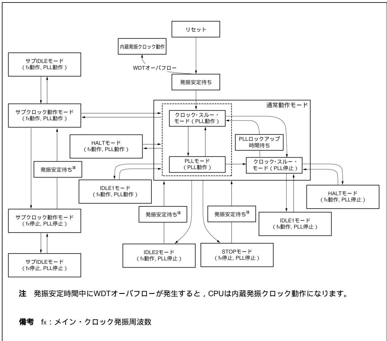
図24 - 1 状態遷移図
