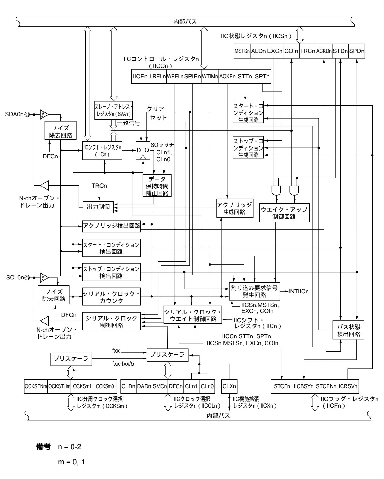
図17-4 I 2 C0nのブロック図
