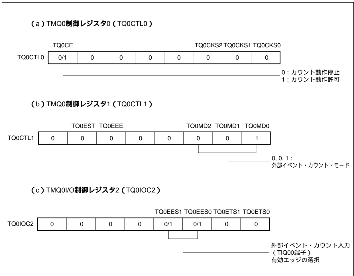
図8 - 15 外部イベント・カウント・モード動作時のレジスタ設定内容(1/2)
