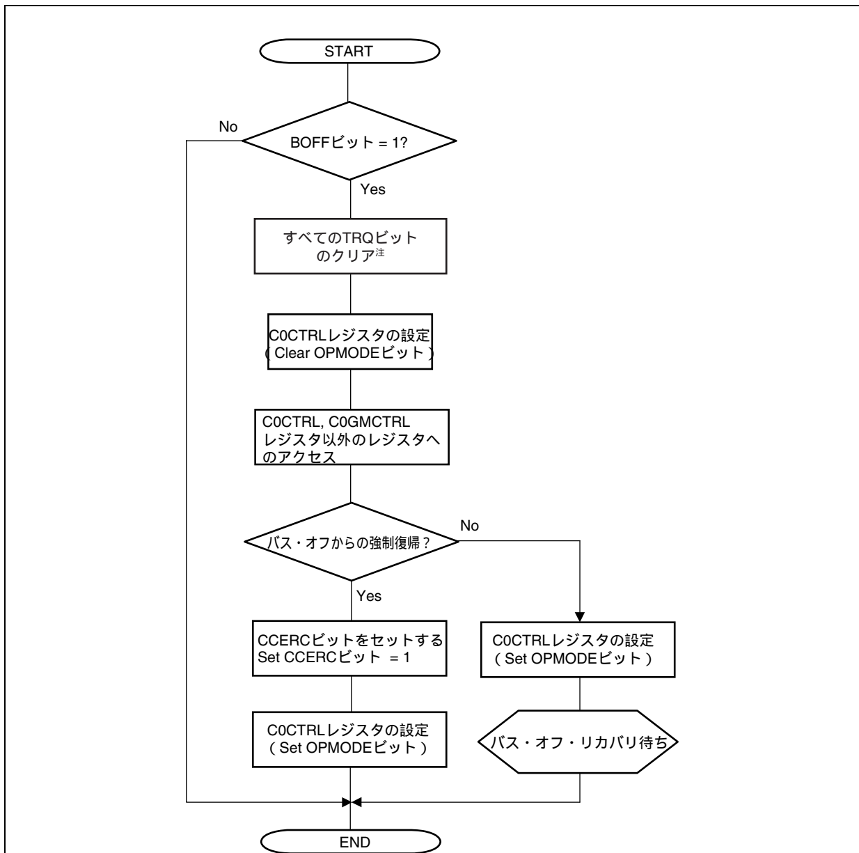
図19 - 54 バス・オフからのリカバリ処理 (ABT付き通常動作モード以外の場合)
