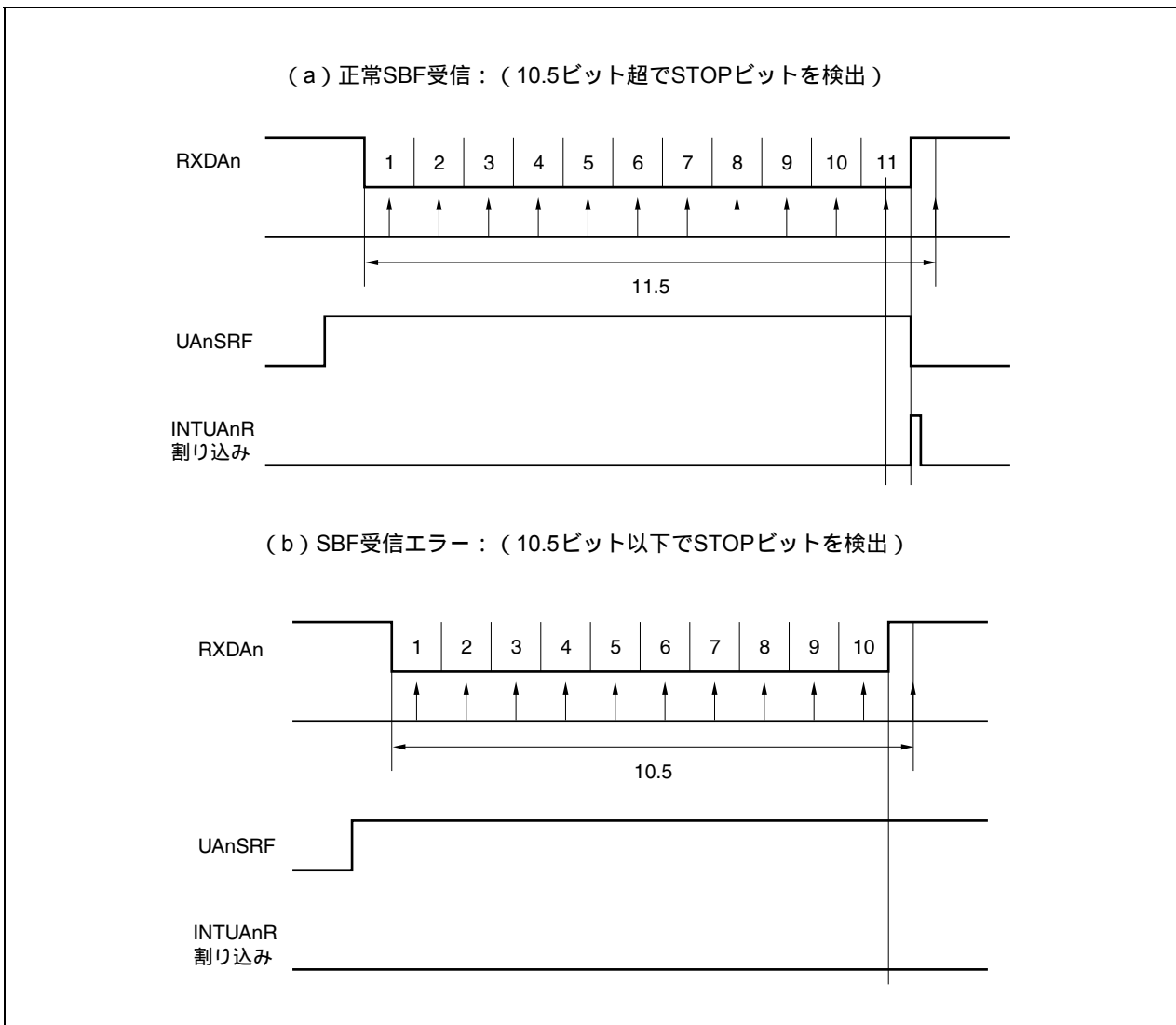
図15 - 9 SBF受信
