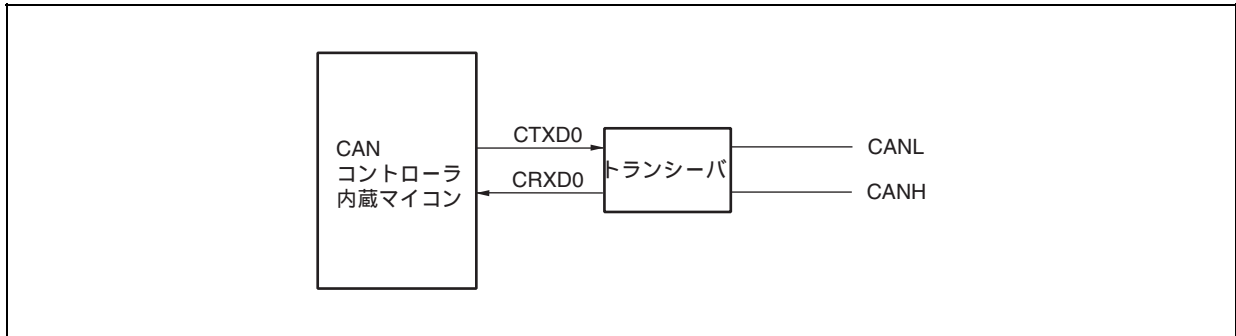
図19 - 22 CANバスへの接続
