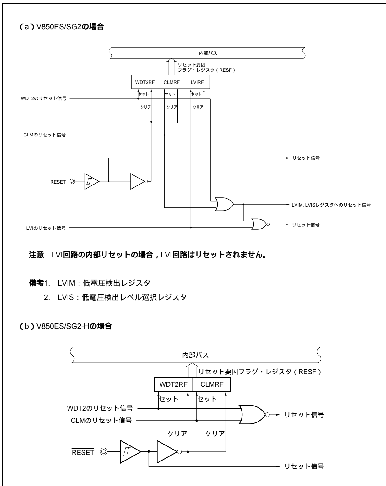
図25 - 1 リセット機能のブロック図
