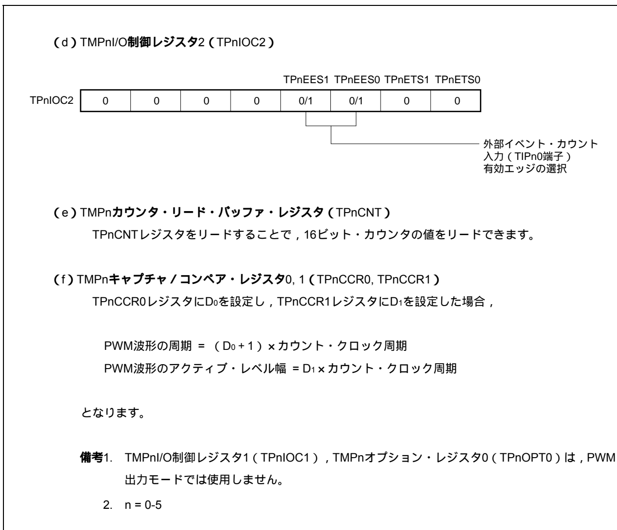
図7 - 30 PWM出力モード動作時のレジスタ設定内容 (2/2)
