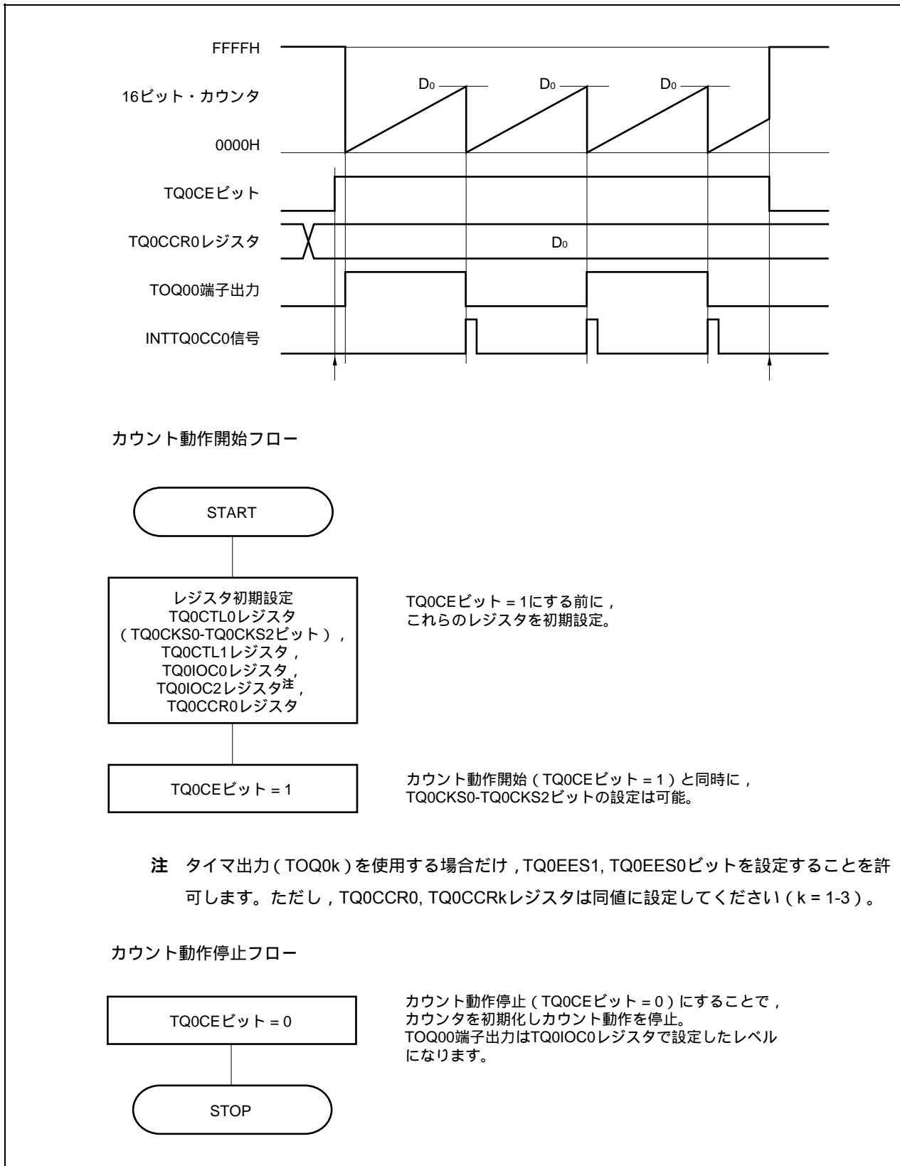
図8-9 インターバル・タイマ・モード使用時のソフトウェア処理フロー
