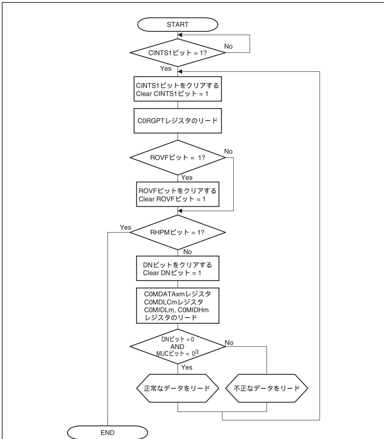
図19 - 51 ソフトウェア・ポーリングによる受信処理
