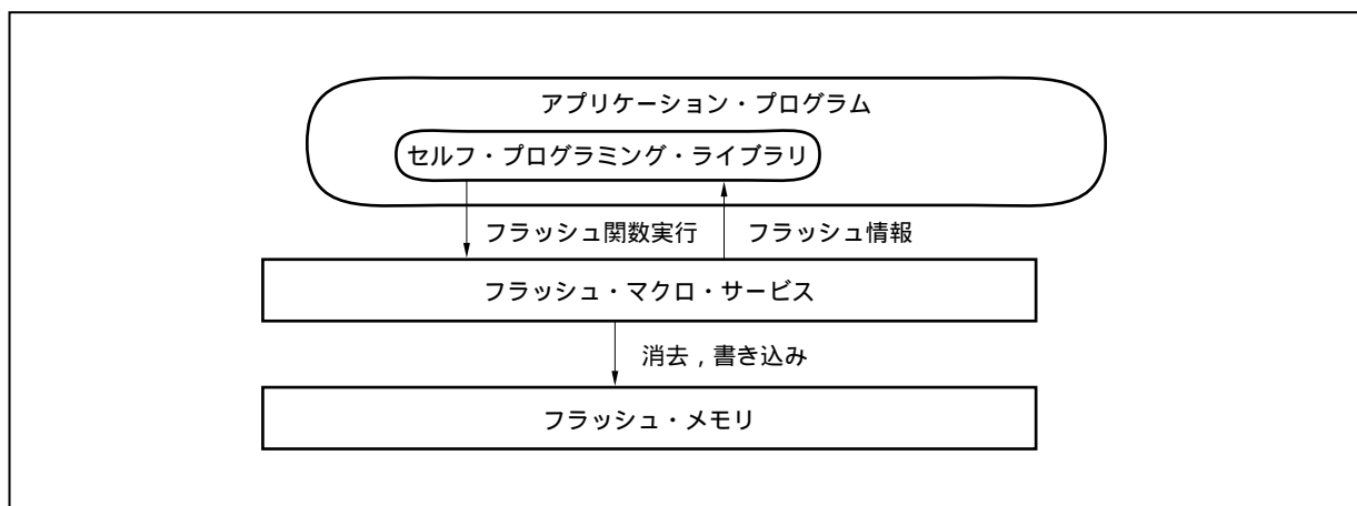
図30 - 16 セルフ・プログラミングの概念図
