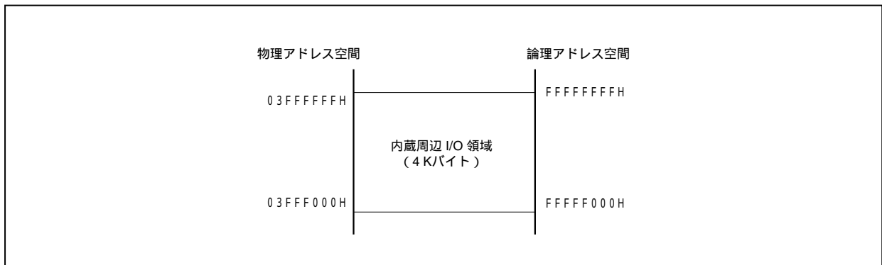
図3 - 13 内蔵周辺I/O領域
