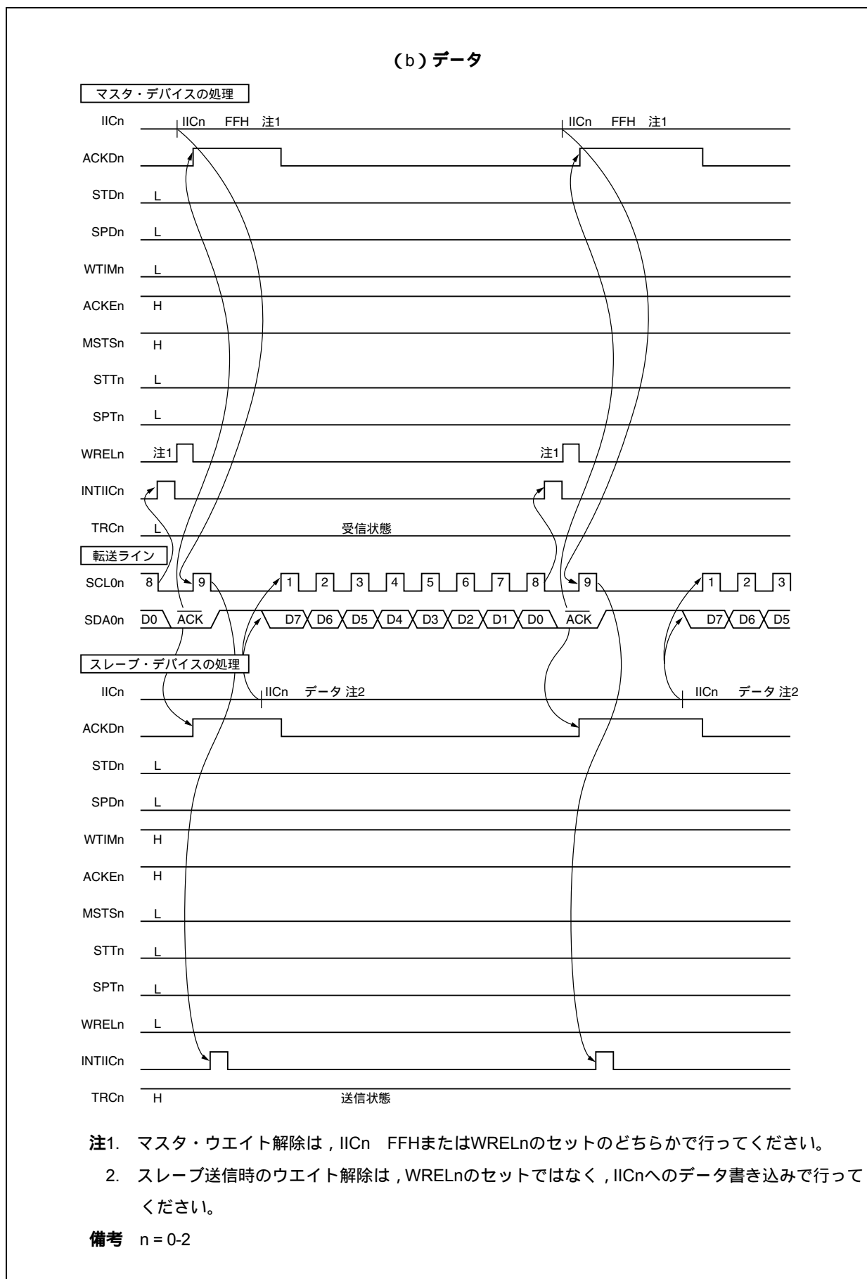
図17-21 スレーブ マスタ通信例 (マスタ:8クロック,スレーブ:9クロックでウエイト選択時) (2/3)
