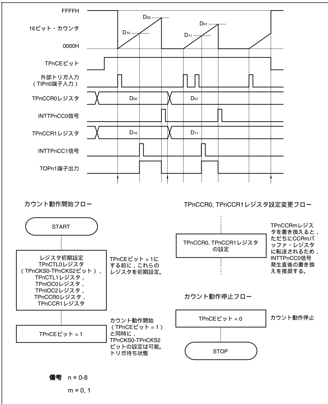
図7-27 ワンショット・パルス出力モード使用時のソフトウェア処理フロー
