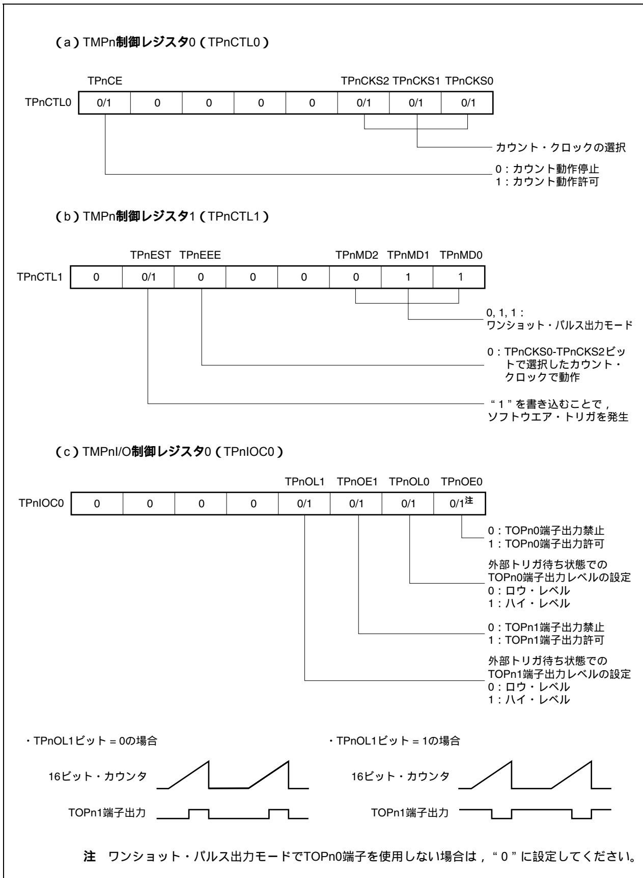
図7-26 ワンショット・パルス出力モード動作時のレジスタ設定内容 (1/2)
