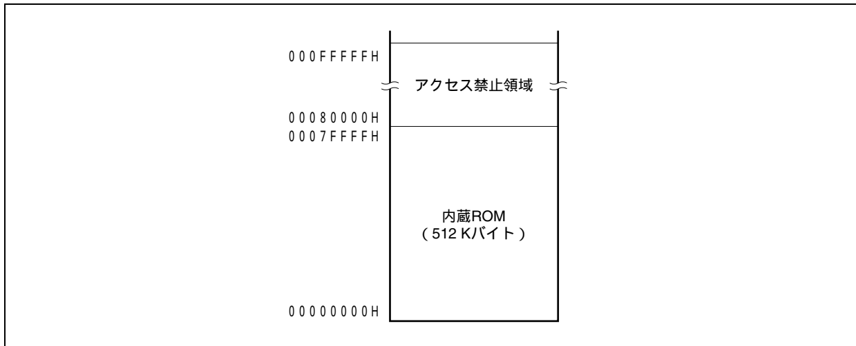
図3 - 5 内蔵ROM領域 (512 Kバイト)
