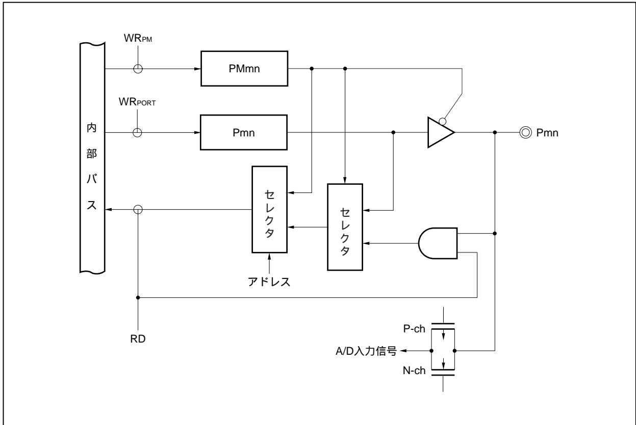
図4-3 タイプA-1のブロック図
