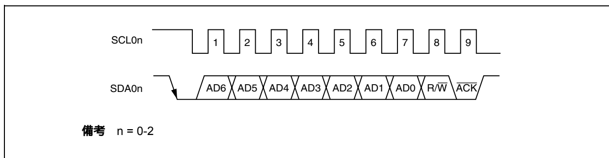
図17-8 アクノリッジ (ACK)
