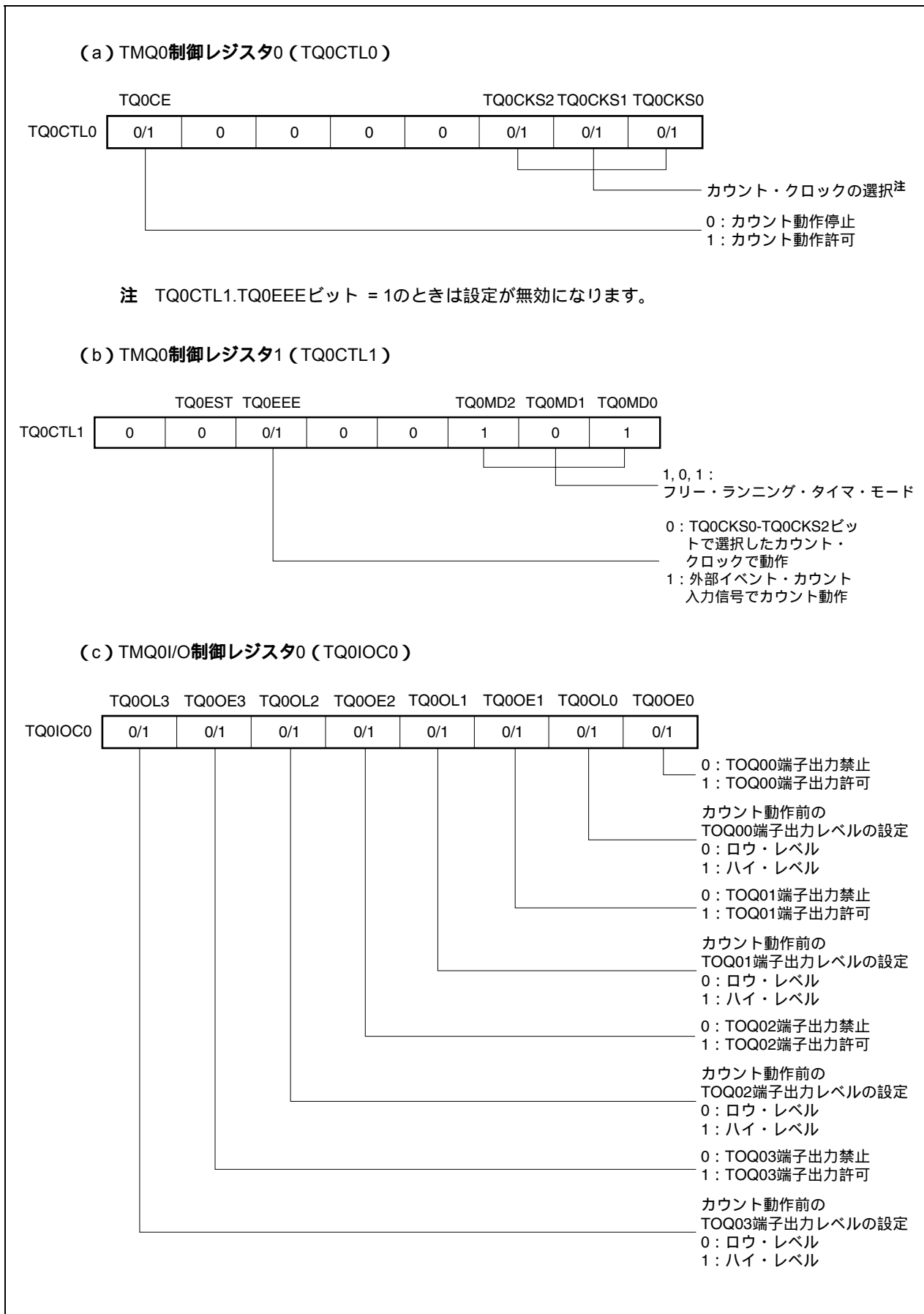
図8 - 35 フリー・ランニング・タイマ・モード動作時のレジスタ設定内容 (1/3)
