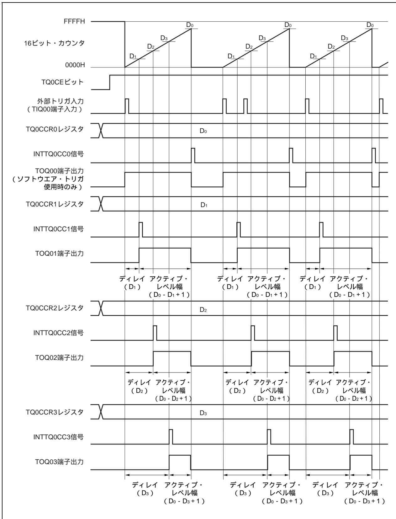
図8 - 25 ワンショット・パルス出力モードの基本タイミング
