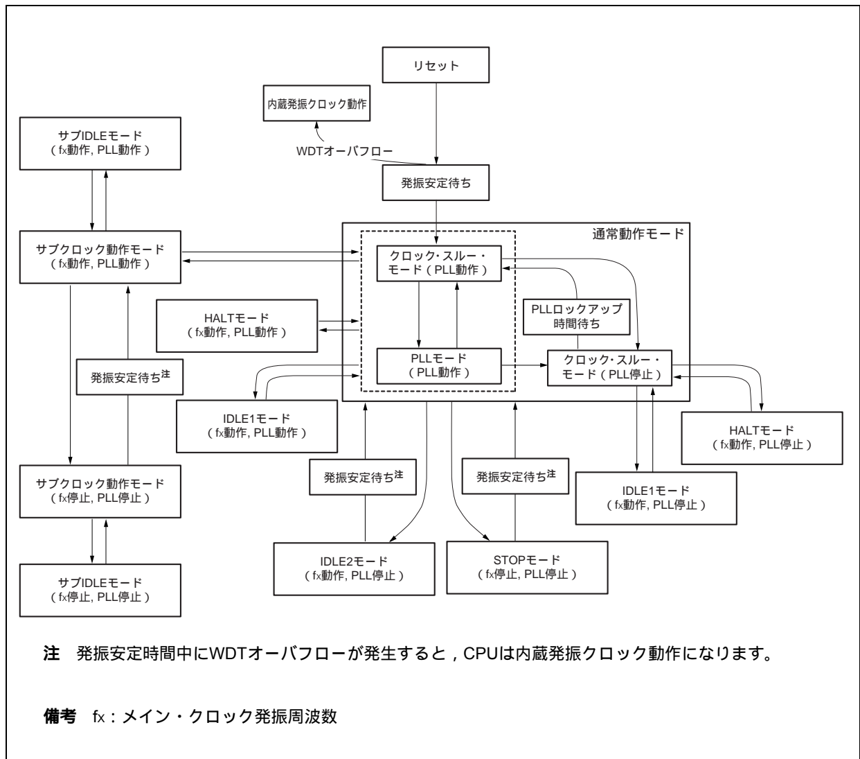
図24 - 1 状態遷移図
