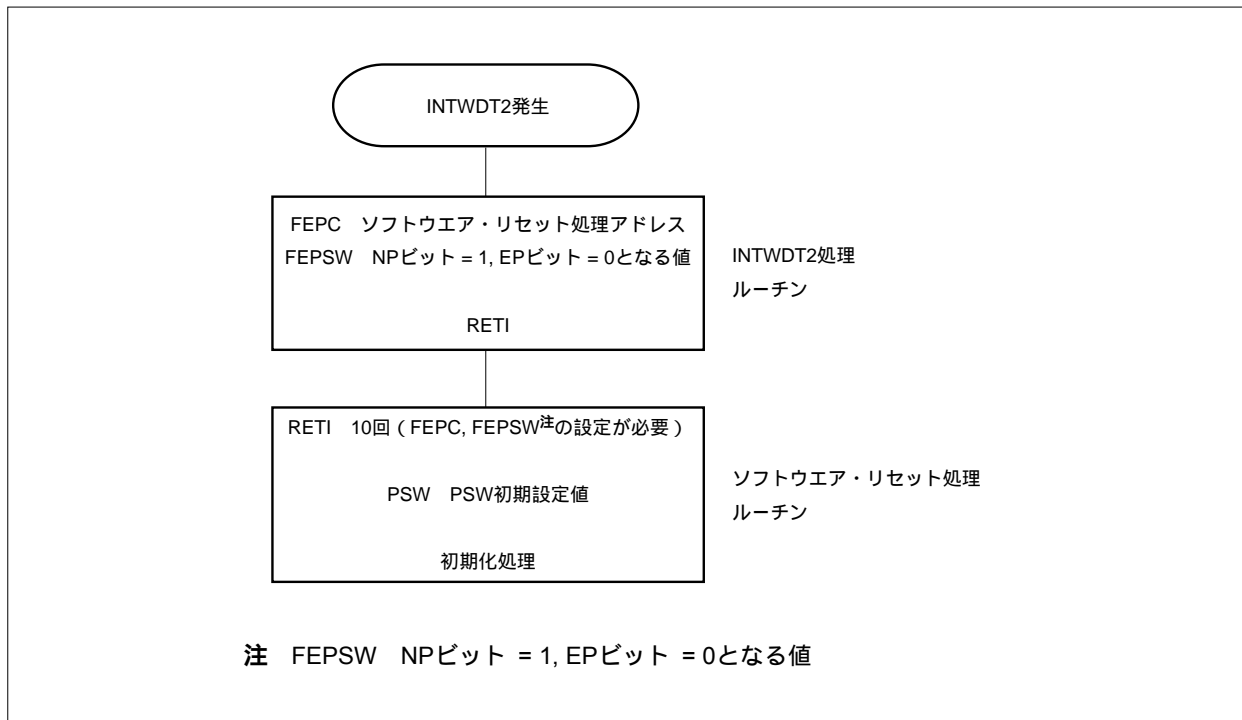
図22 - 4 ソフトウェア・リセット処理
