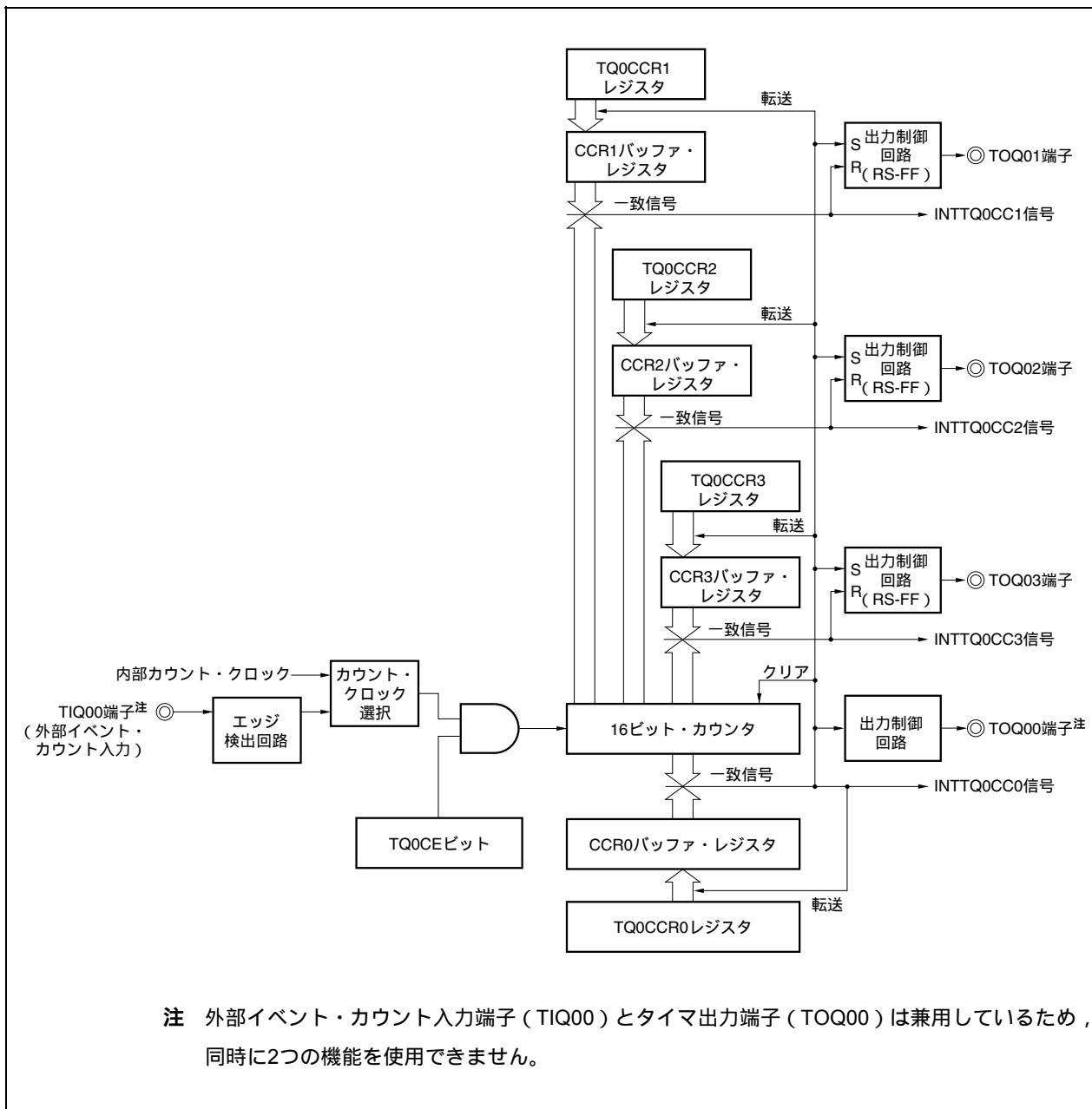
図8 - 28 PWM出力モードの構成図
