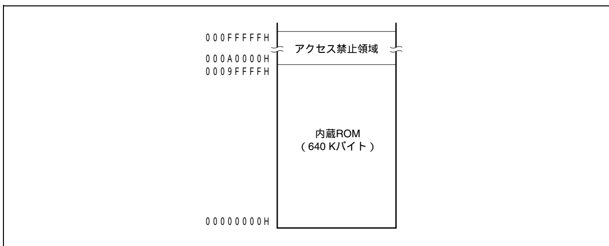
図3 - 6 内蔵ROM領域 (640 Kバイト)
