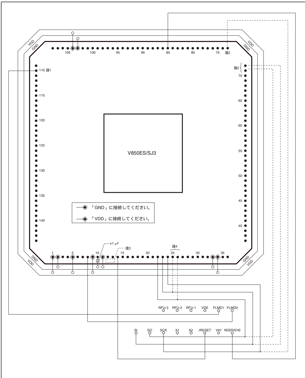
図30 - 6 V850ES/SJ3フラッシュ書き込み用アダプタ(FA-144GJ-UEN-A)の配線例(CSIB0+HSモード時)(1/2)
