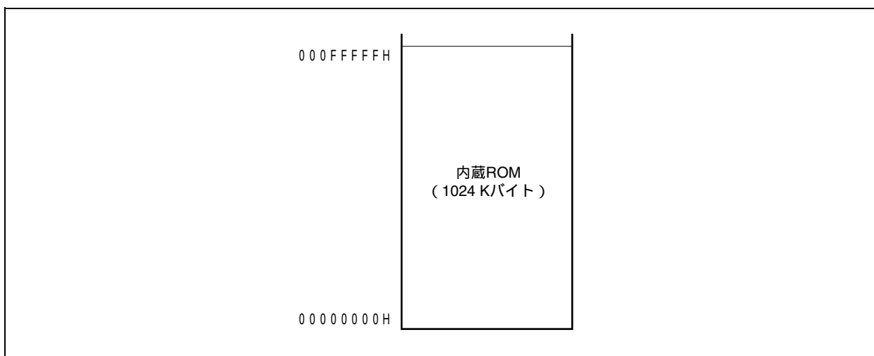
図3 - 8 内蔵ROM領域 (1024 Kバイト)
