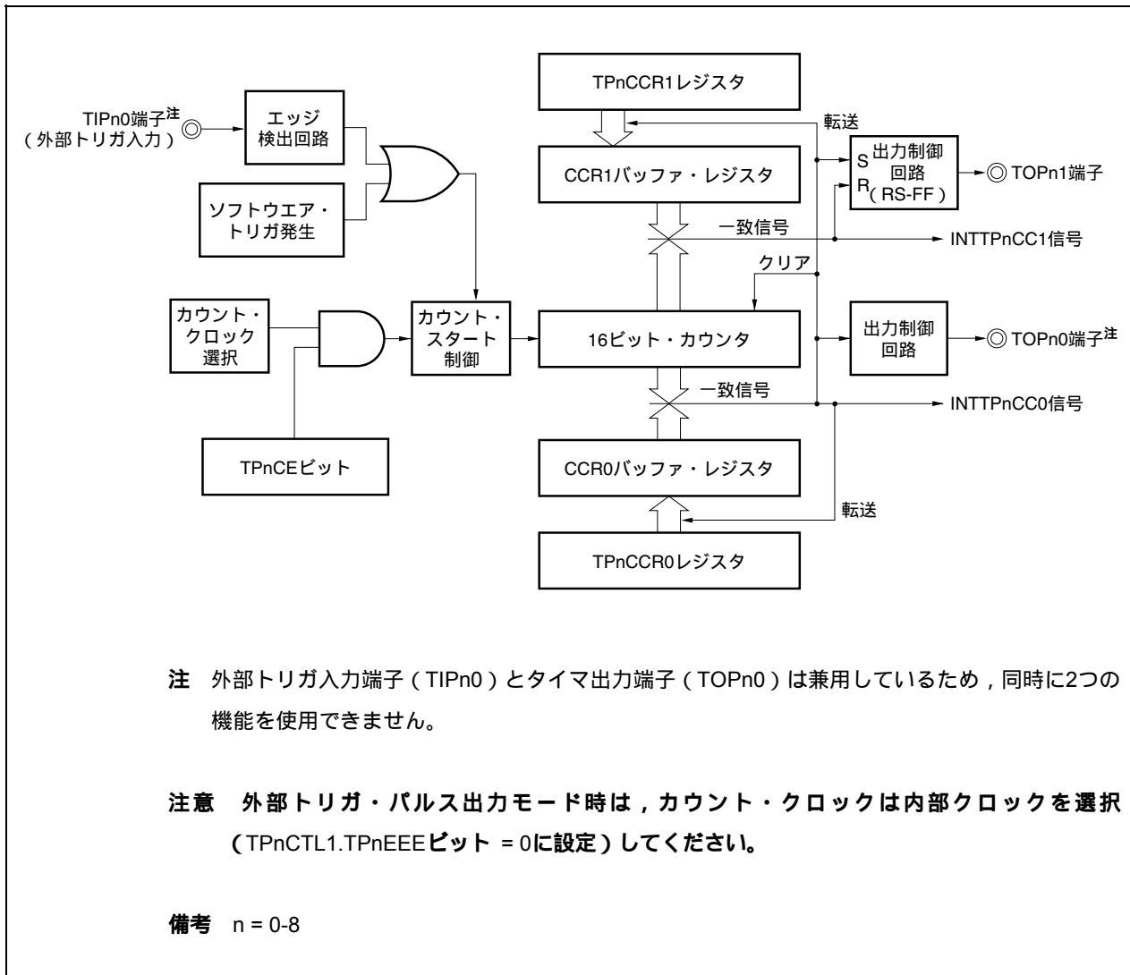
図7 - 20 外部トリガ・パルス出力モードの構成図
