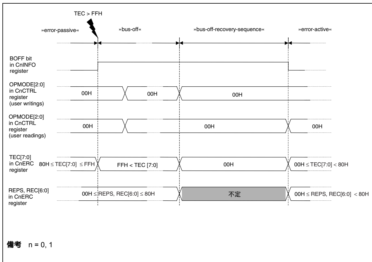
図19 - 17 通常リカバリ・シーケンスによるバス・オフからの復帰動作
