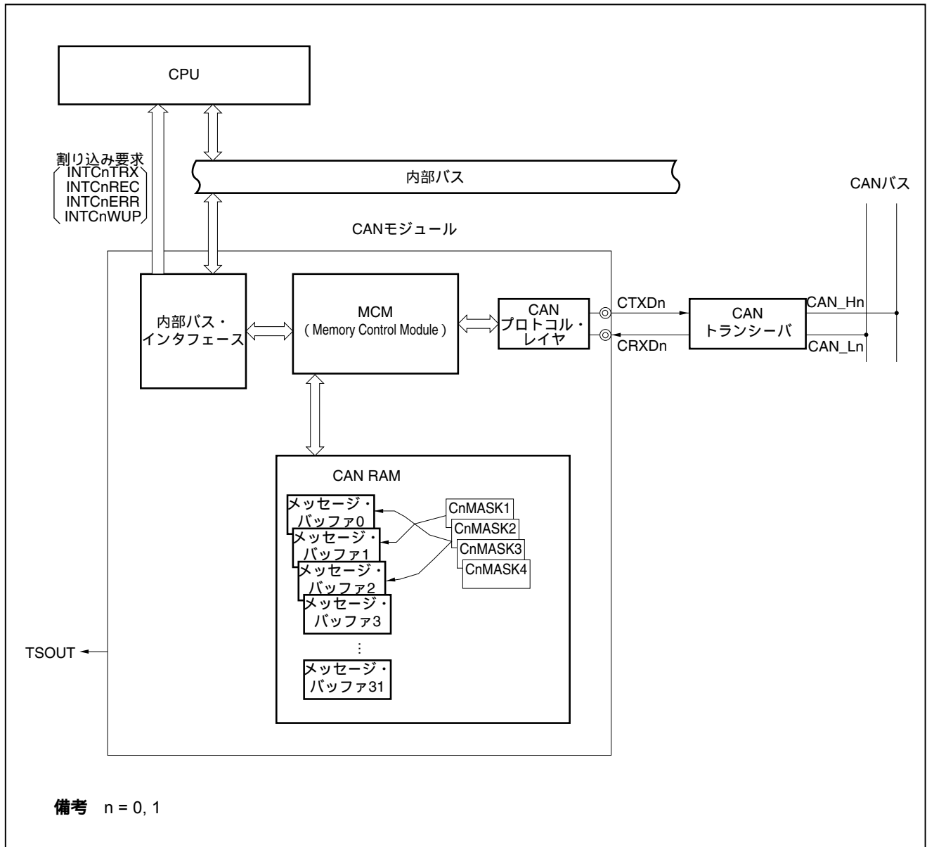
図19 - 1 CANのブロック図
