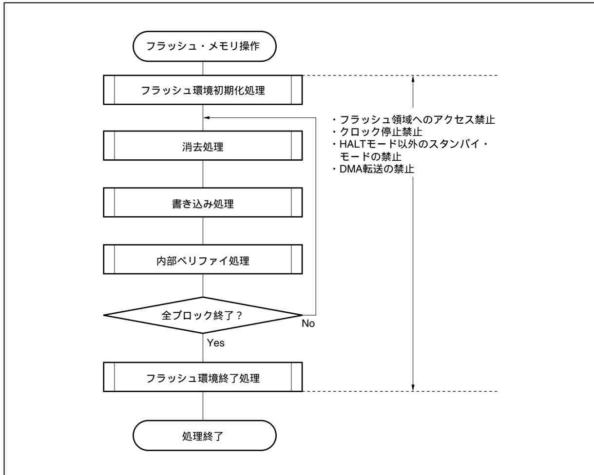
図30 - 17 標準セルフ・プログラミング・フロー
