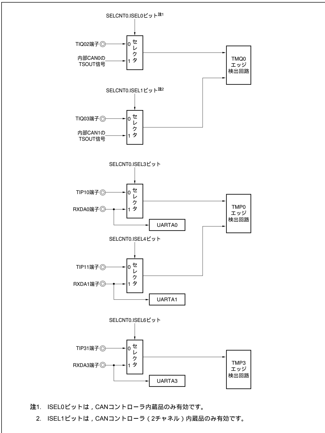
図7 - 42 セレクト機能のブロック図
