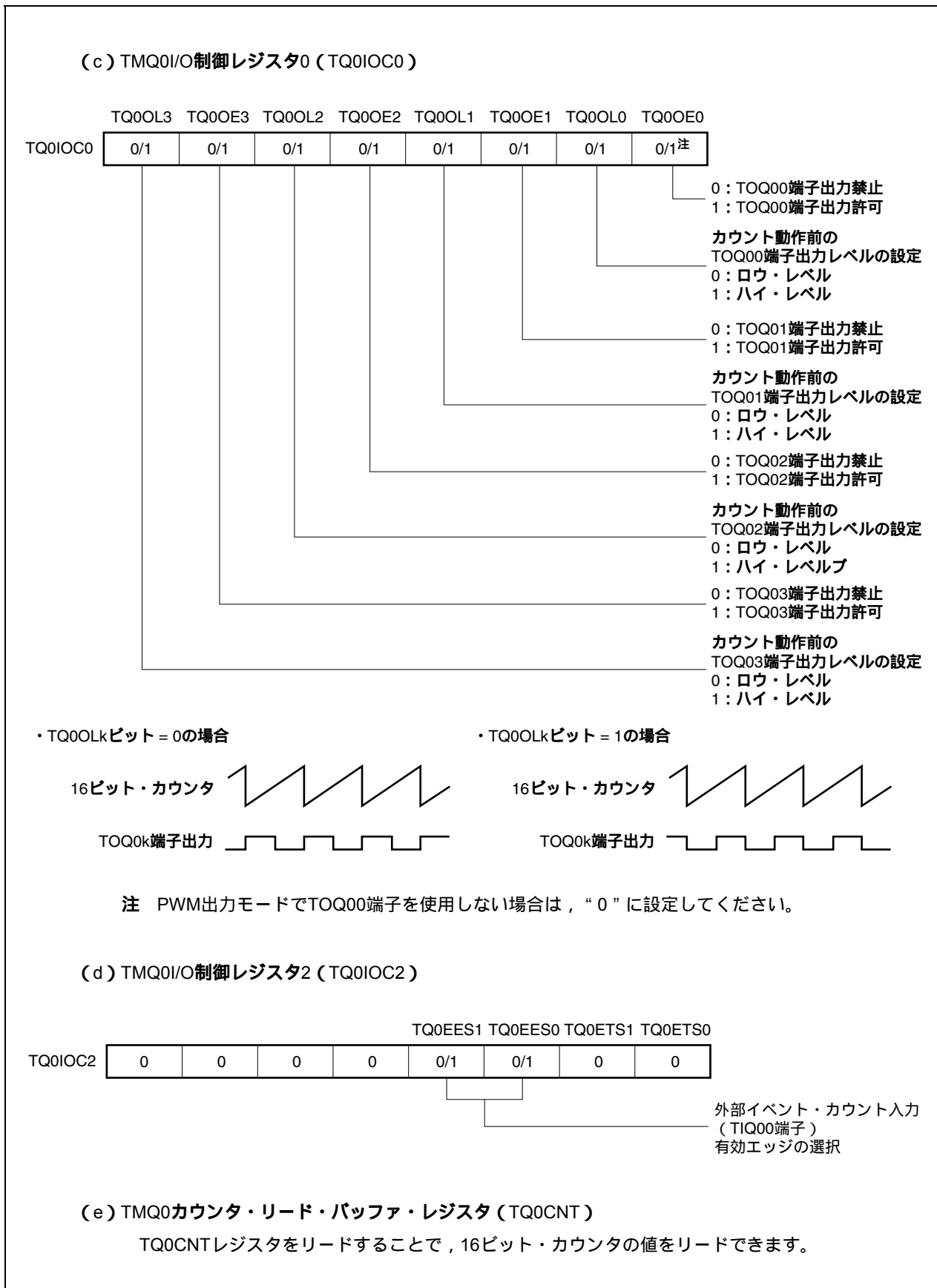
図8 - 30 PWM出力モード動作時のレジスタ設定内容 (2/3)
