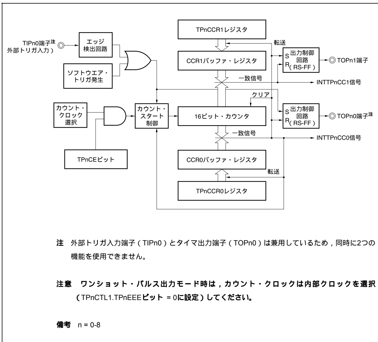
図7-24 ワンショット・パルス出力モードの構成図
