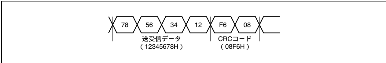
図21 - 4 CRC送信例
