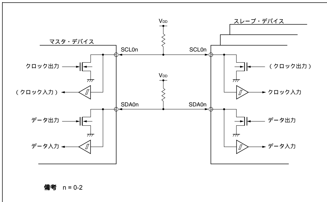
図17-3 端子構成図
