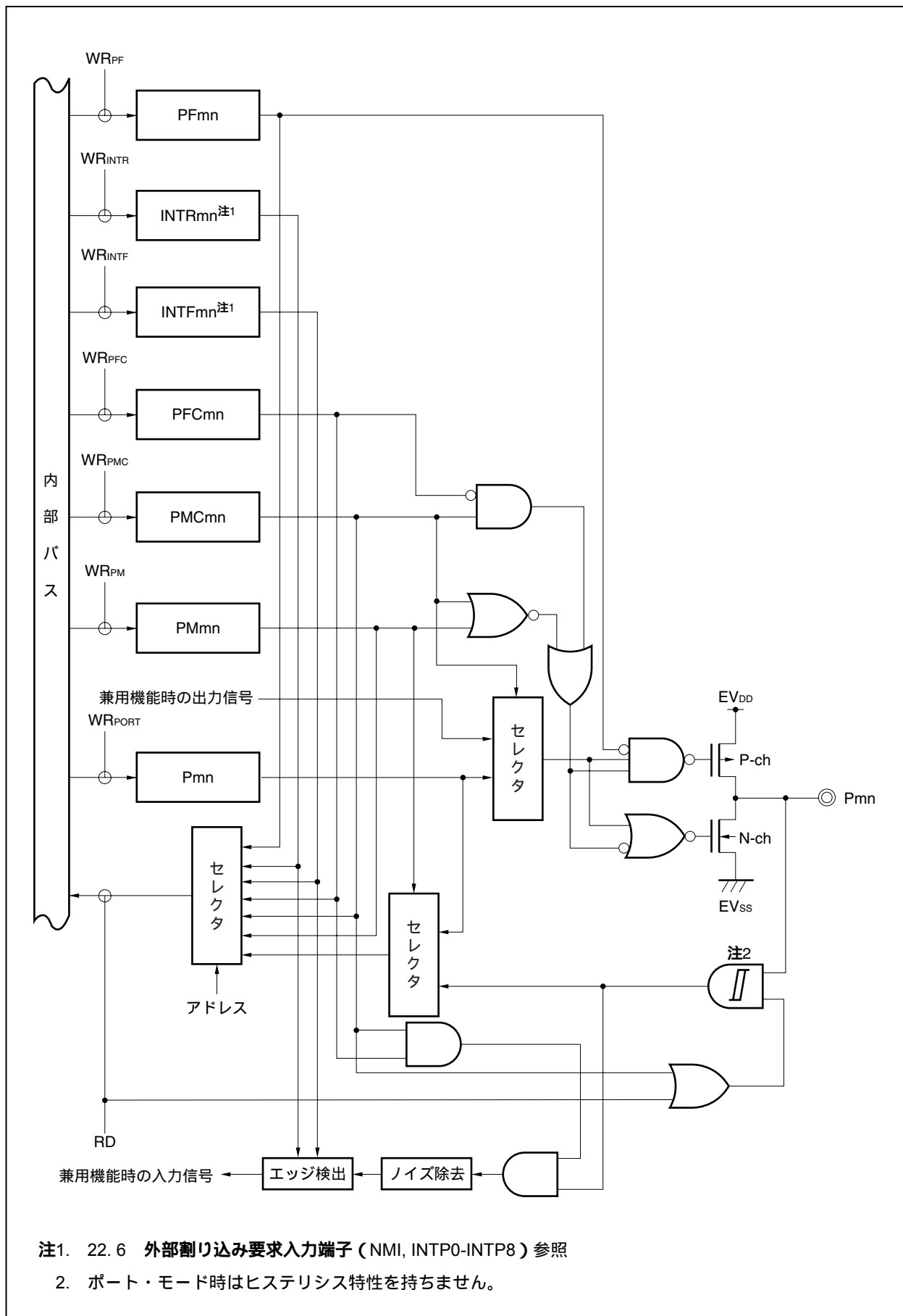
図4-23 タイプN-2のブロック図
