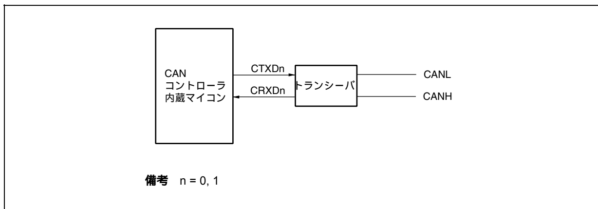
図19 - 22 CANバスへの接続
