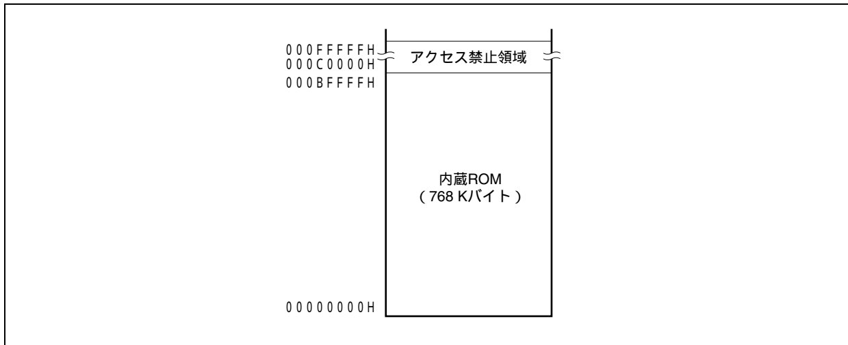
図3 - 7 内蔵ROM領域 (768 Kバイト)
