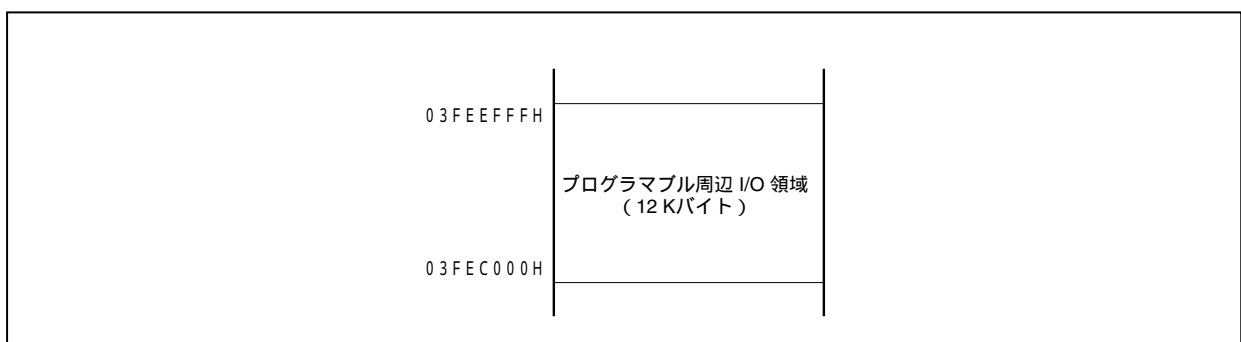
図3 - 14 プログラマブル周辺I/O領域
