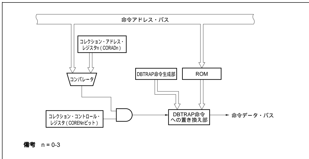
図29 - 1 ROMコレクションのブロック図
