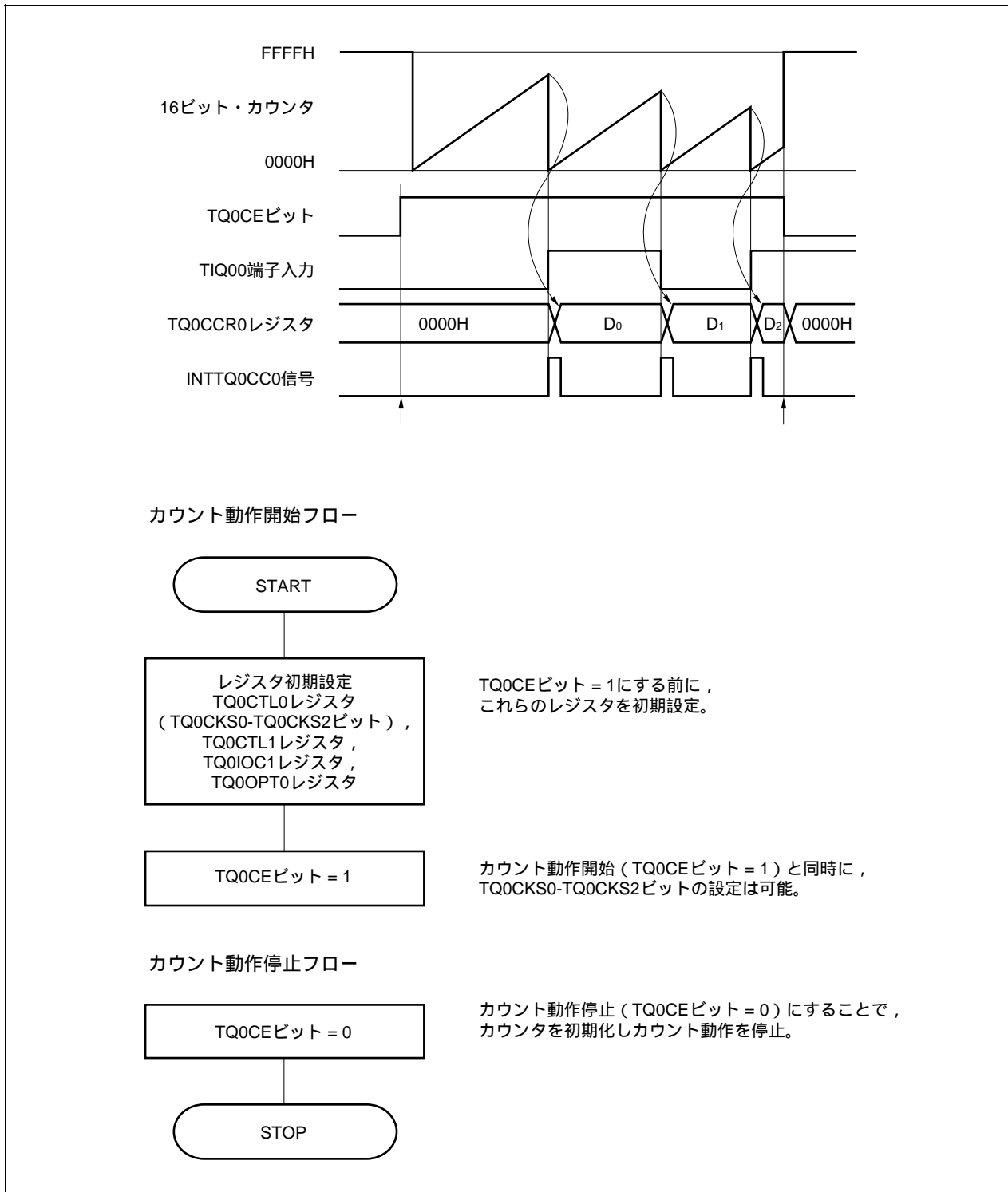
図8 - 41 パルス幅測定モード使用時のソフトウェア処理フロー
