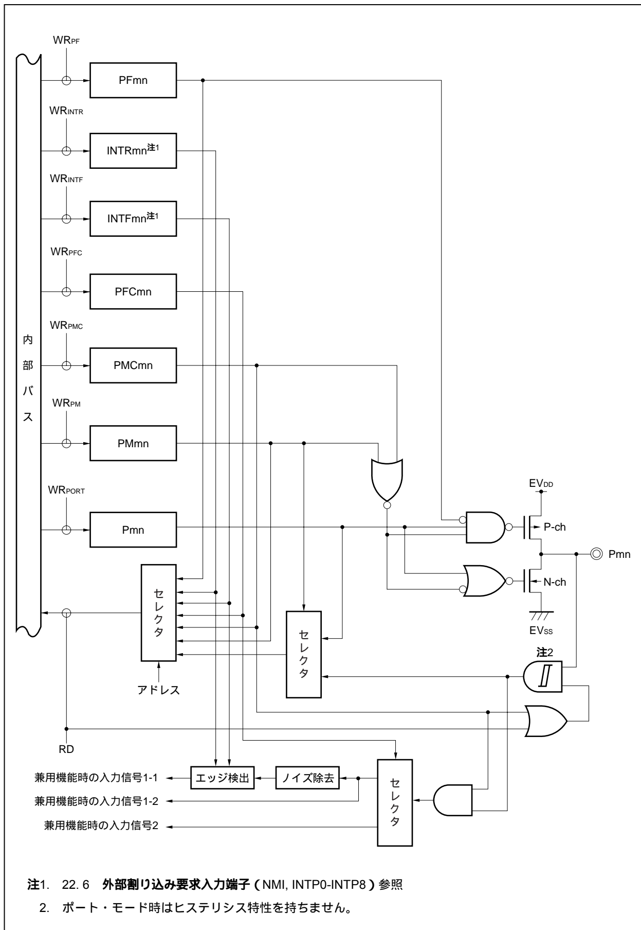
図4-24 タイプN-3のブロック図
