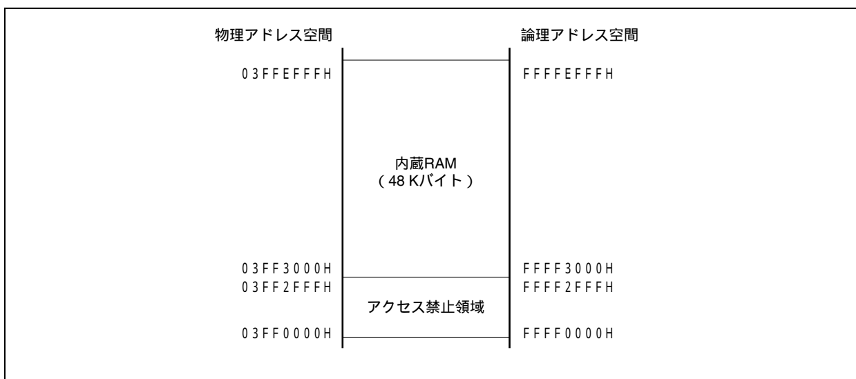
図3 - 11 内蔵RAM領域 (48 Kバイト)
