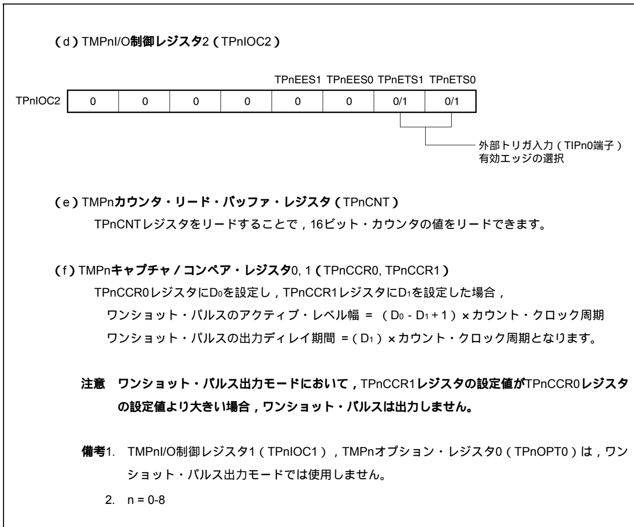
図7-26 ワンショット・パルス出力モード動作時のレジスタ設定内容 (2/2)
