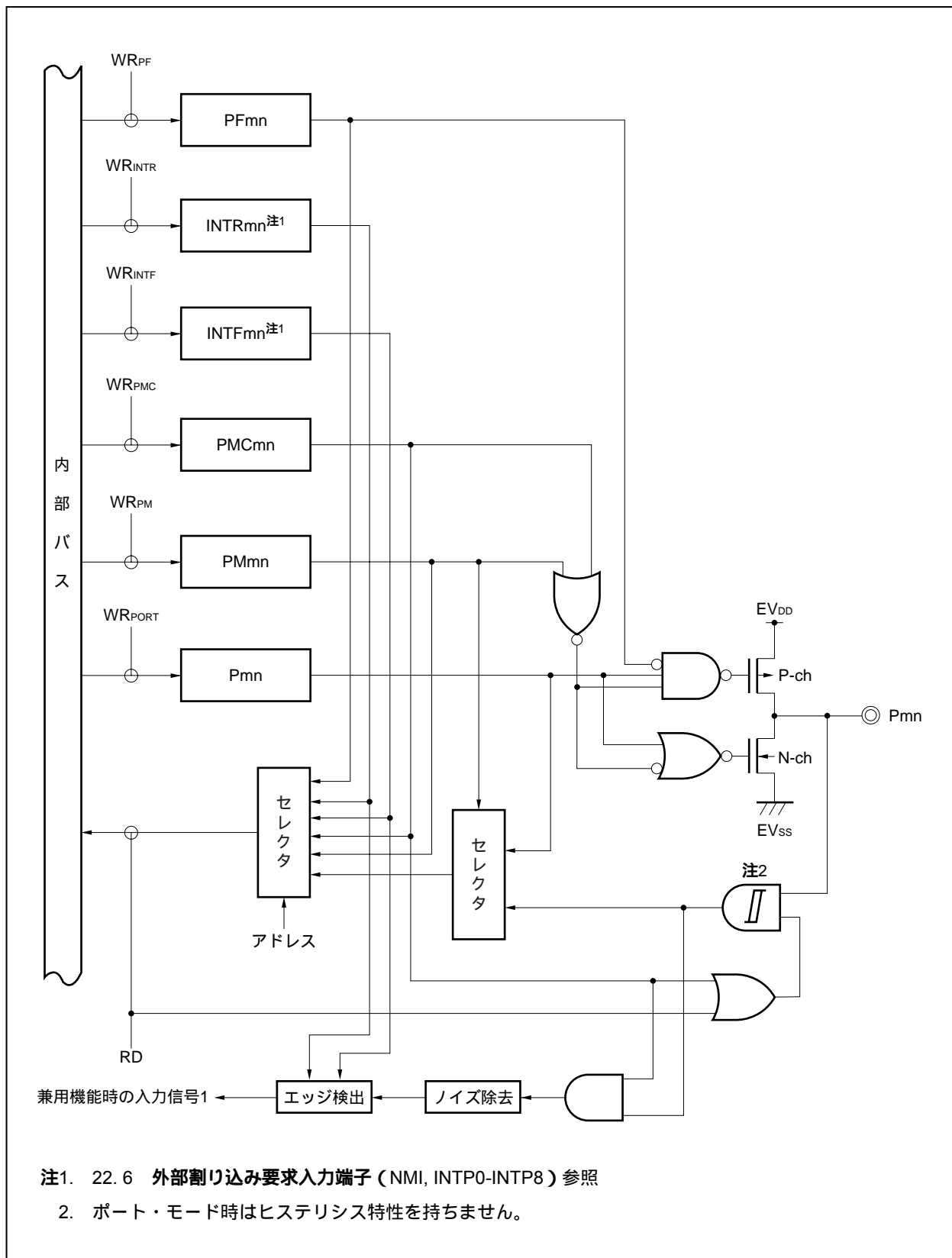
図4-20 タイプル-1のブロック図
