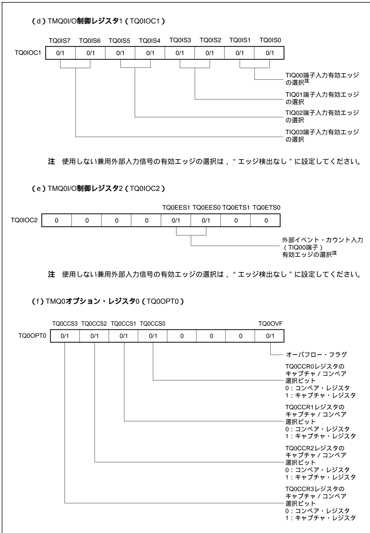
図8 - 35 フリー・ランニング・タイマ・モード動作時のレジスタ設定内容 (2/3)
