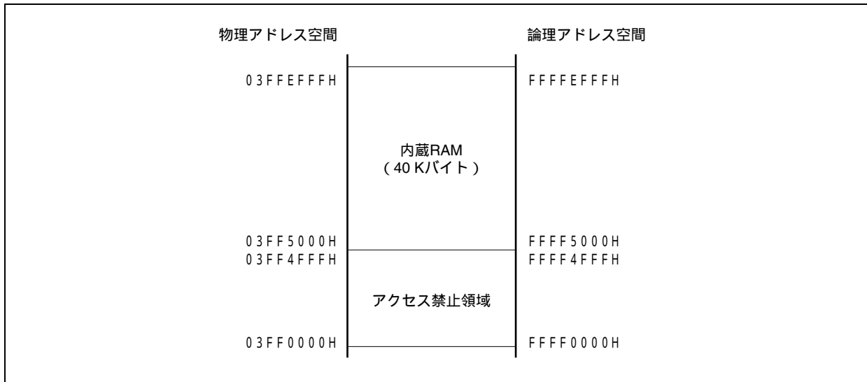
図3 - 10 内蔵RAM領域 (40 Kバイト)
