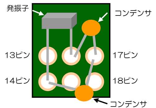
78K0/KF2用評価ボード接続図
