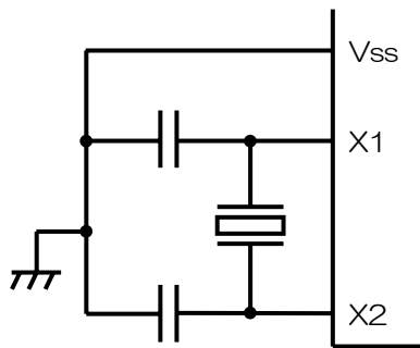
発振回路
