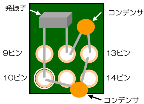
78K0/KE2用評価ボード接続図
