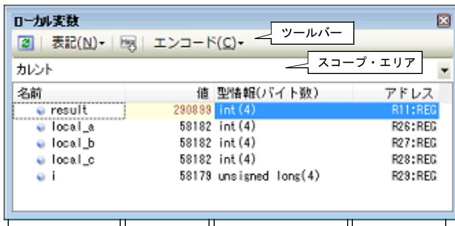
図 2.51 ローカル変数の内容の表示（ローカル変数パネル）
