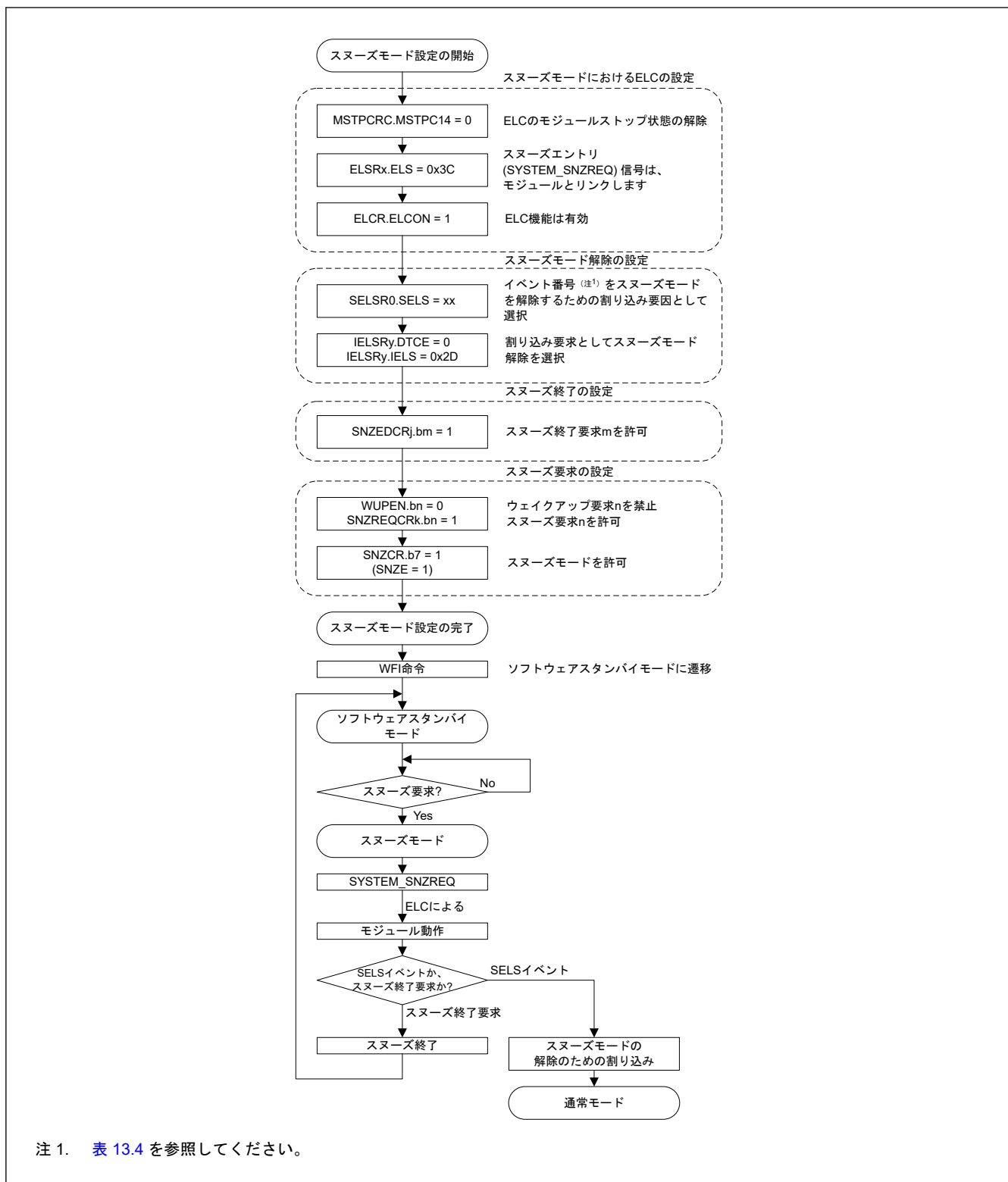
図 10.9 スヌーズモードで ELC を使用するための設定例
