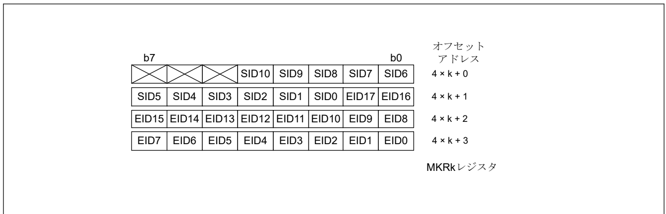
図 29.14 マスクレジスタの構造 ( j = 0 \sim 7 )
