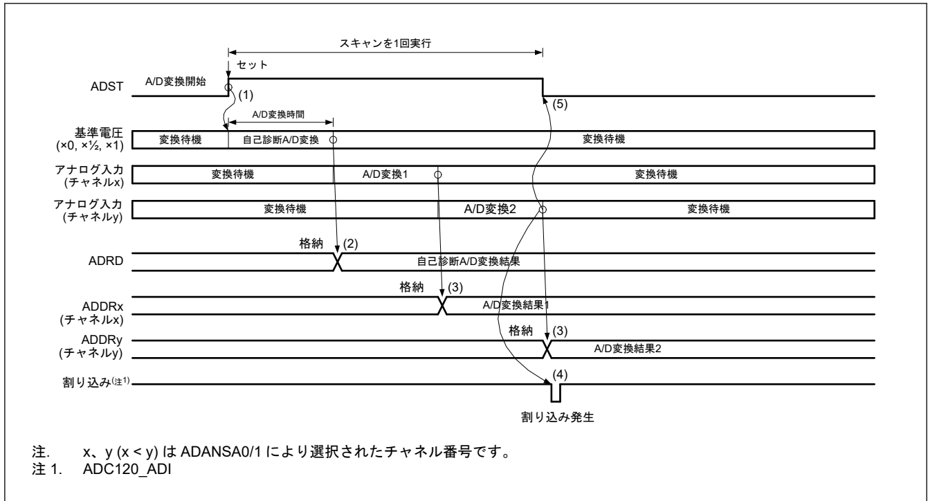
図 37.8 シングルスキャンモードの基本動作例 (アナログ入力 (チャンネル x、y) 選択+自己診断)
