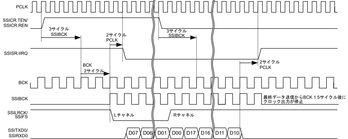
図 32.34 BCKASTP ビットの動作例 (BCKASTP = 1 での通信動作の場合)
