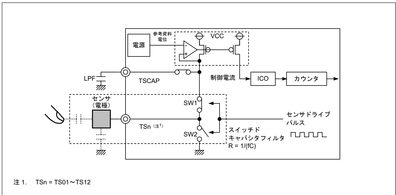
図 40.4 計測部回路
