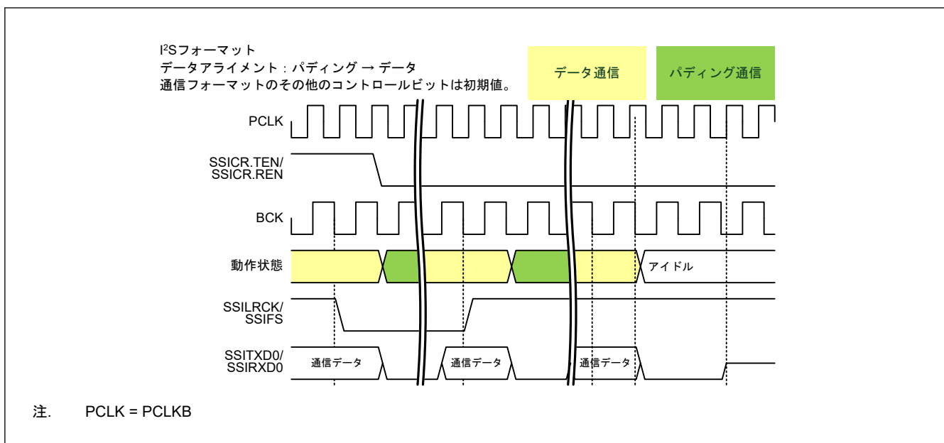
図 32.49 データ通信からの停止（パディングビットあり）
