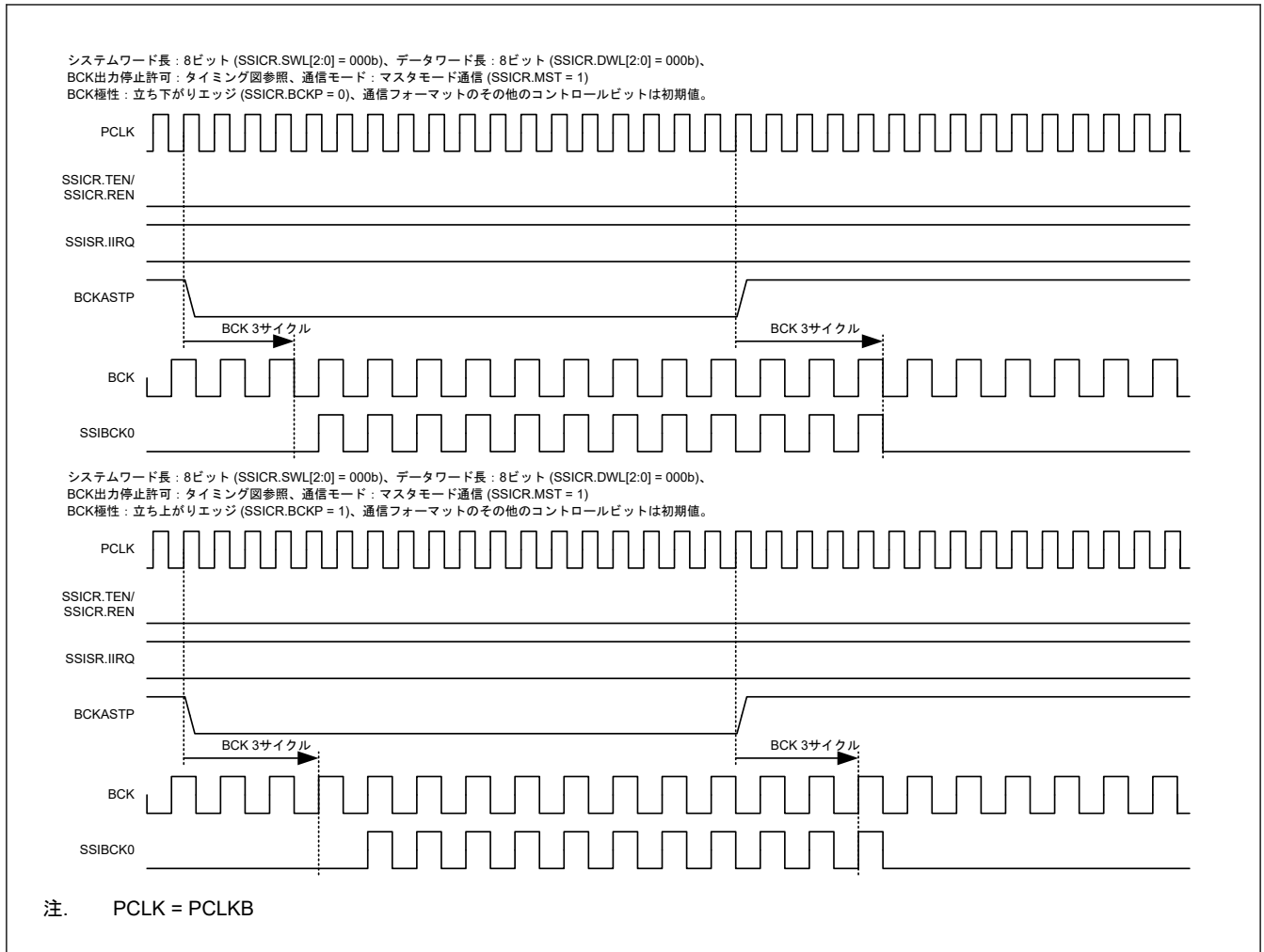
図 32.33 BCKASTP ビットの動作例 (アイドル状態の場合)
