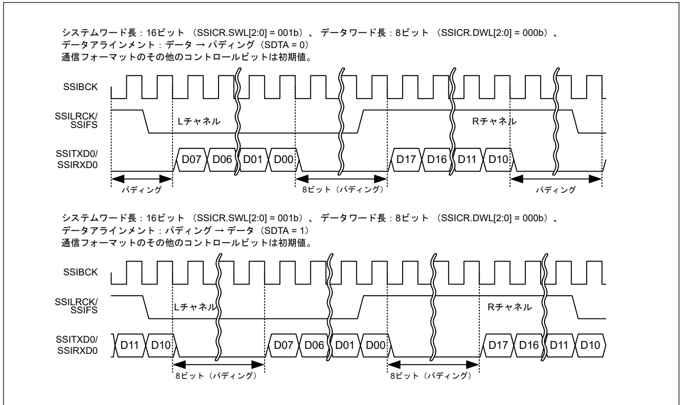
図 32.9 パディングビットを伴うシリアルデータのアライメント設定
