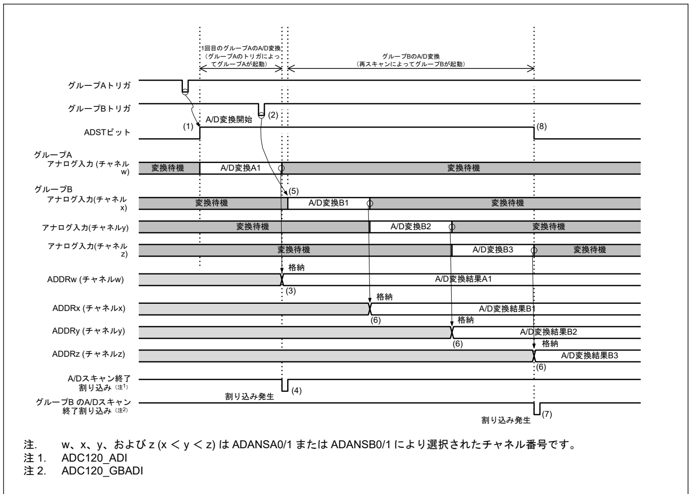
図 37.20 グループ優先動作の例 1-3 : グループ A スキャン中のグループ B トリガ入力、再スキャンあり (ADGSPCR.GBRSCN = 1、ADGSPCR.GBRP = 0、および ADGSPCR.LGRRS = 0 の場合)
