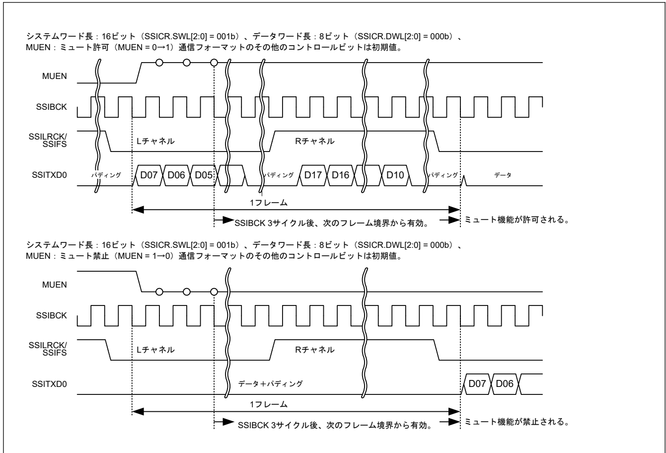
図 32.4 ミュート機能設定時のデータ送信
