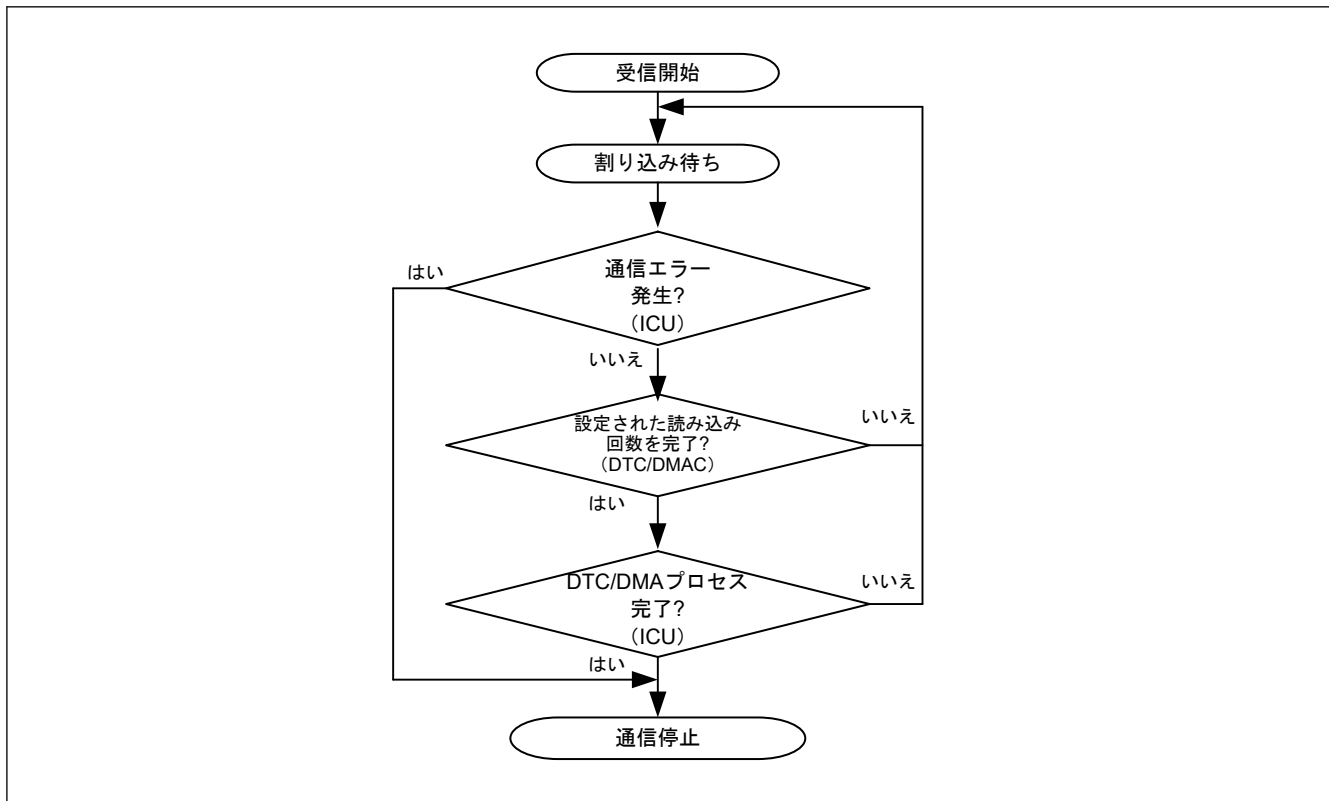
図 32.54 受信手順
