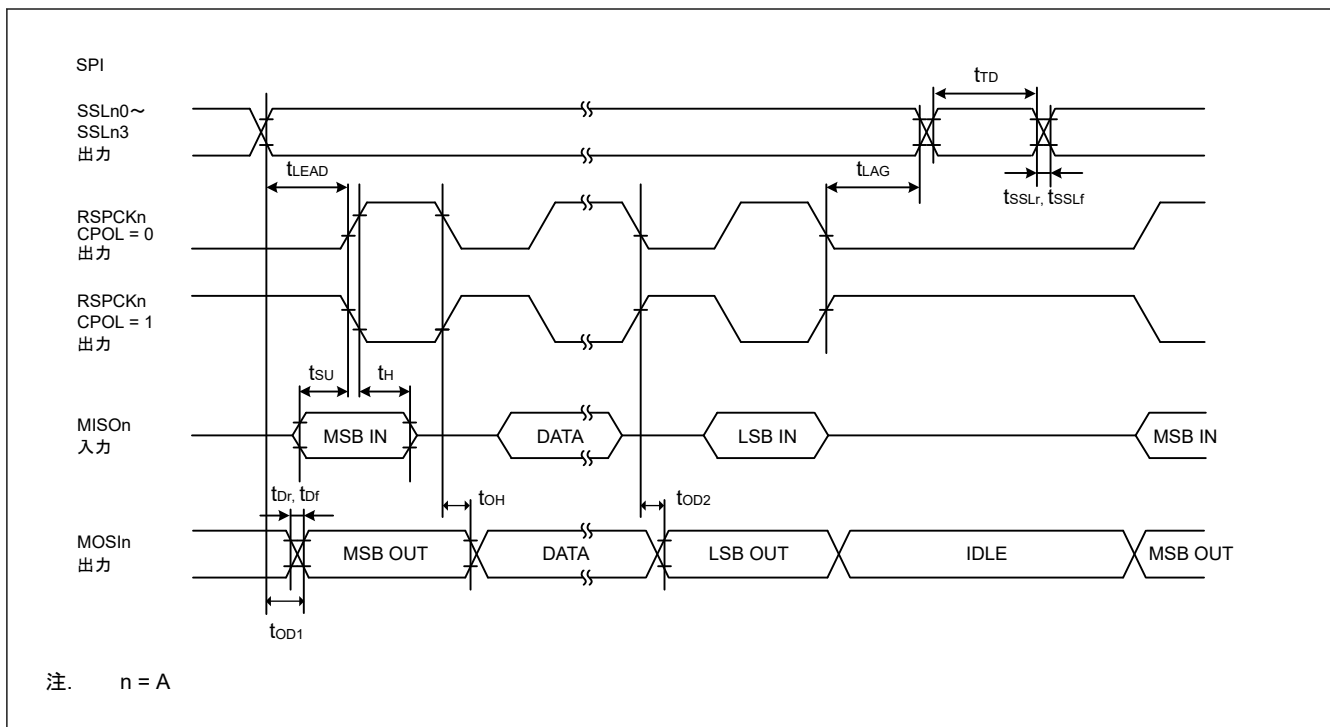
図 47.35 CPOL = 0 の場合におけるマスタの SPI タイミング
