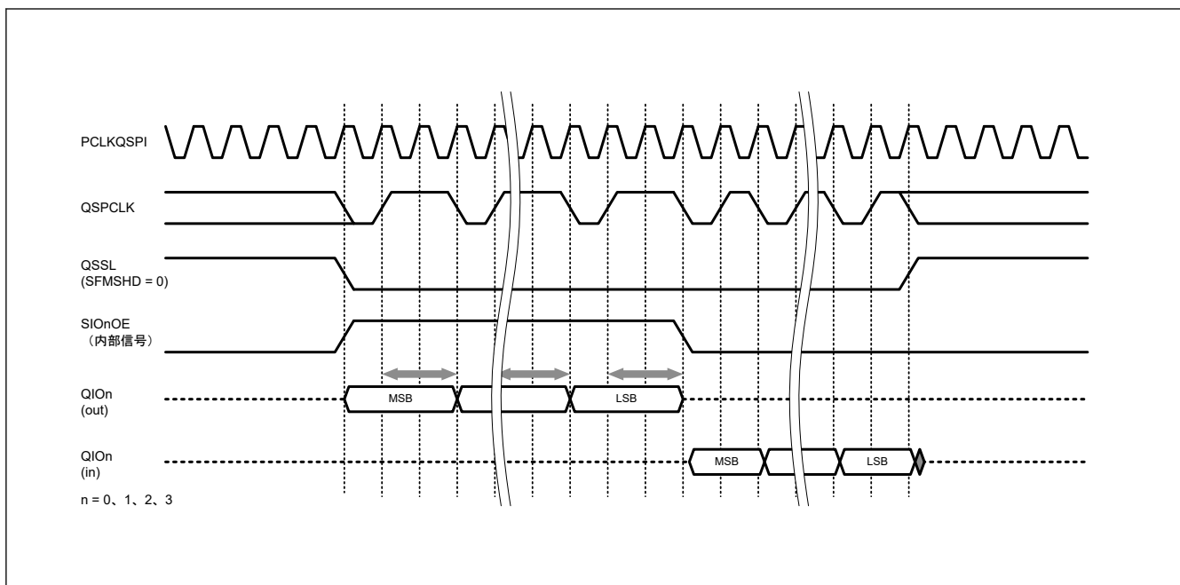
図 31.16 SFMSMD.SFMOSW ビットを使用したシリアルデータ出力のホールド時間調整
