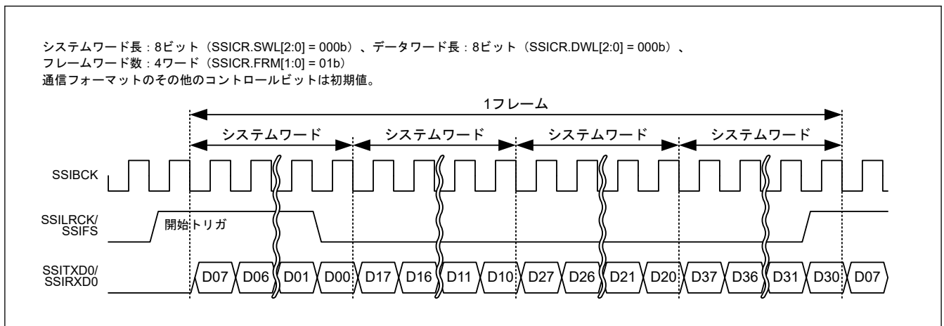
図 32.40 TDM フォーマット (パディングなし、システムワード長 = データワード長)
