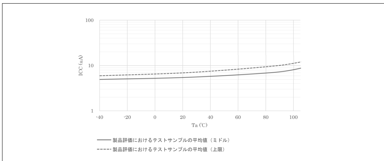
図 47.5 ディープソフトウェアスタンバイモード時の温度依存性、SRAM および USB レジューム検出部への電源供給なし、パワーオンリセット回路、低消費電力機能有効（参考データ）
