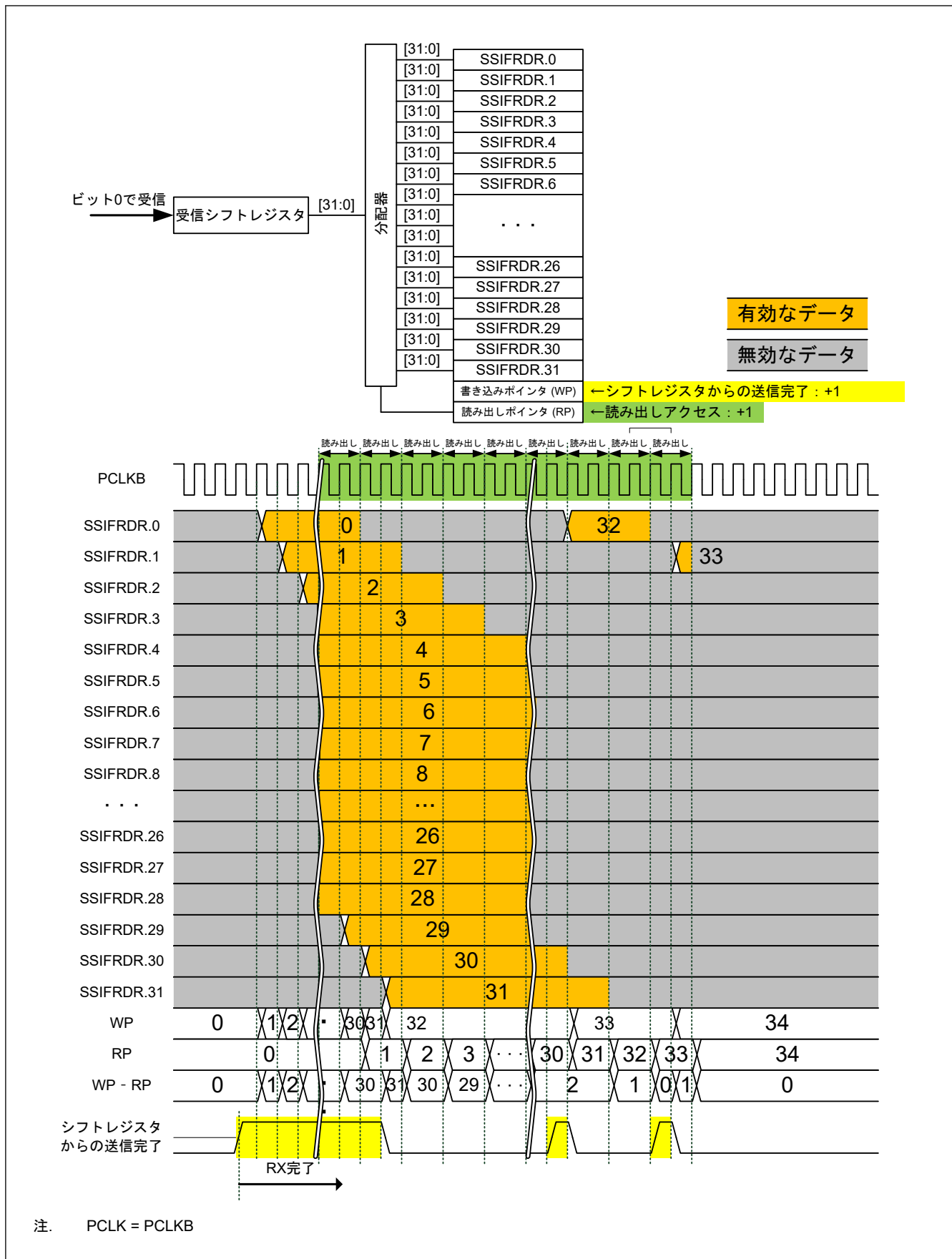
図 32.31 受信 FIFO データレジスタと受信シフトレジスタの構成、および FIFO の動作例
