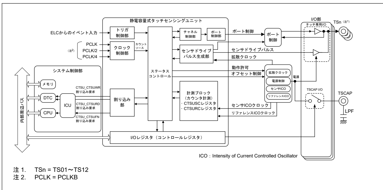
図 40.3 CTSUS ブロック図
