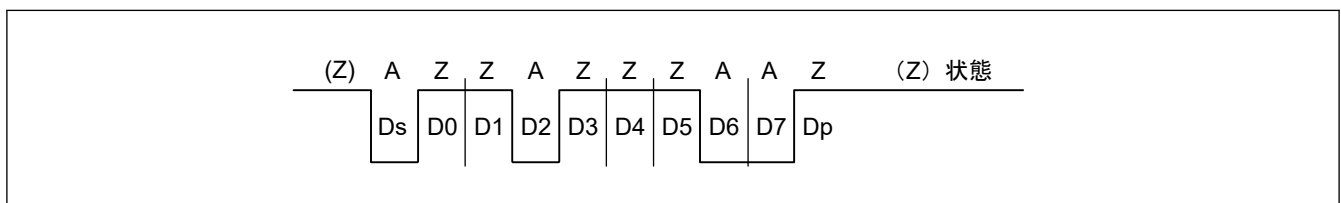
図 27.79 ダイレクトコンベンション (SCMR.SDIR ビット = 0、SCMR.SINV ビット = 0、SMR_SMCI.PM ビット = 0)
