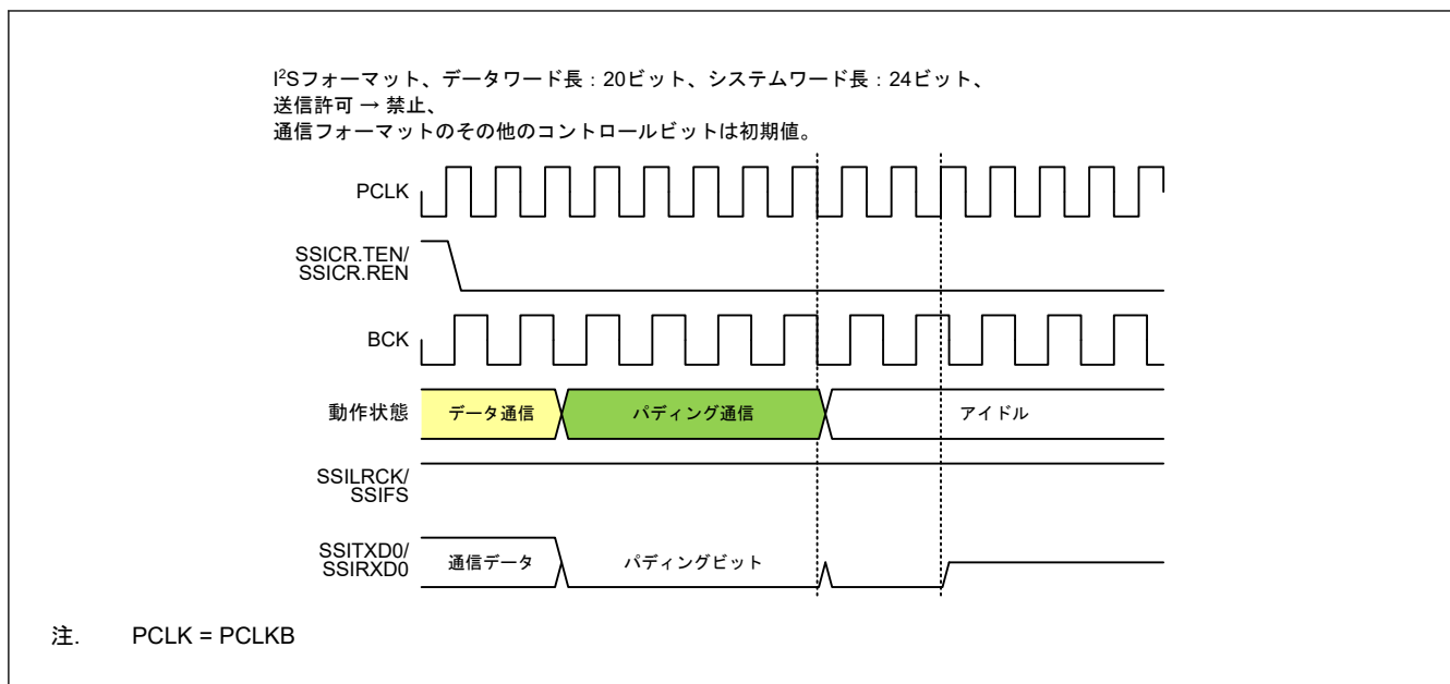
図 32.50 パディング通信からの停止
