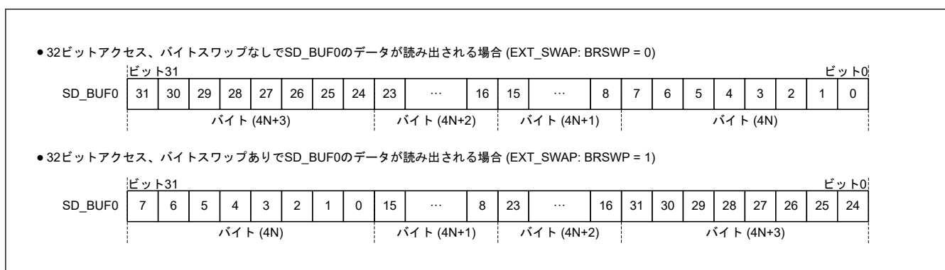
図 33.5 SD_BUF0 からの読み出し
