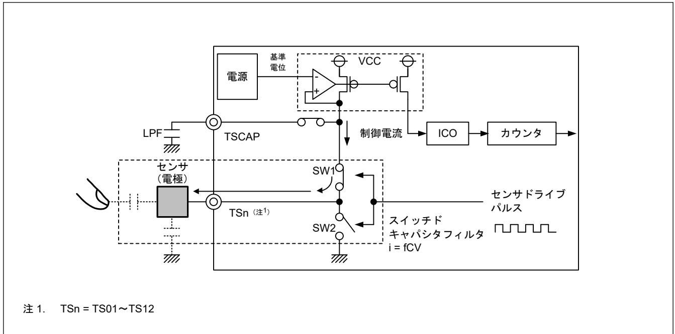
図 40.5 充電動作
