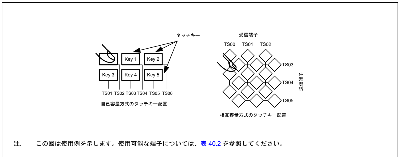
図 40.8 自己容量方式と相互容量方式の概要
