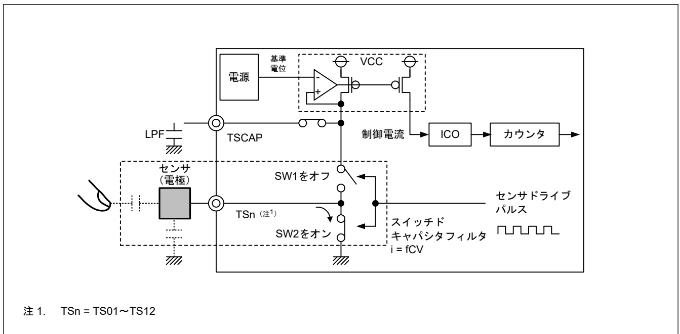
図 40.6 放電動作
