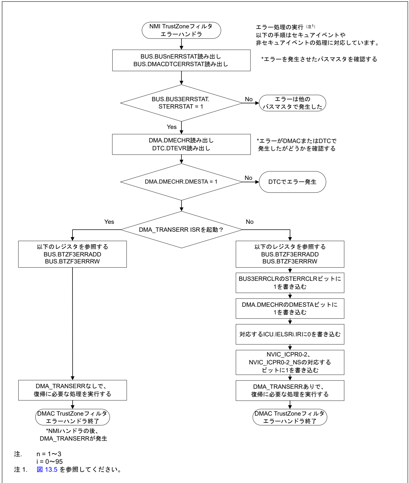
図 16.25 スレーブ TrustZone フィルタエラーの NMI ハンドラにおける処理
