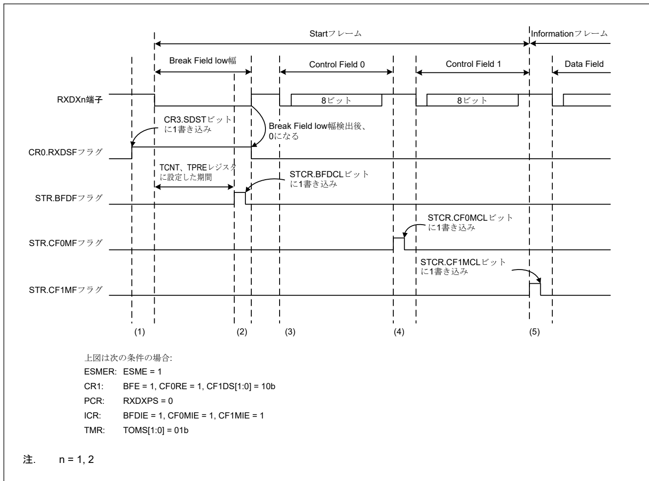
図 27.106 Start Frame 受信時の動作例
