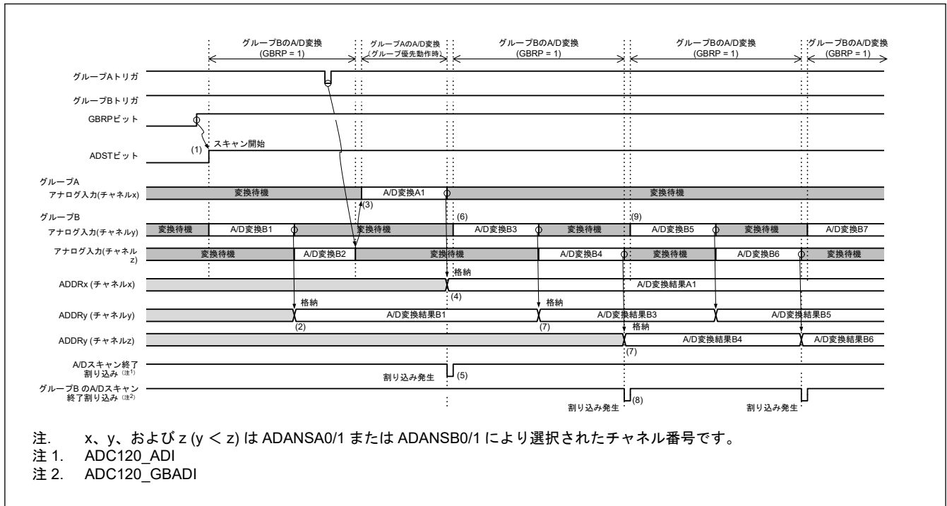
図 37.22 グループ優先動作の例 1-5 : グループ B のシングルスキャン連続動作 (ADGSPCR.GBRP = 1、ADGSPCR.LGRRS = 0 の場合)
