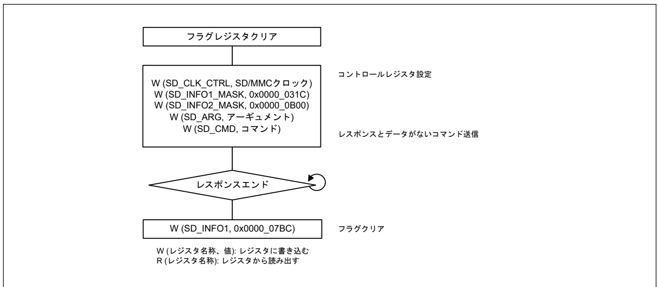
図 33.8 レスポンスまたはデータがないコマンドのフロー例
