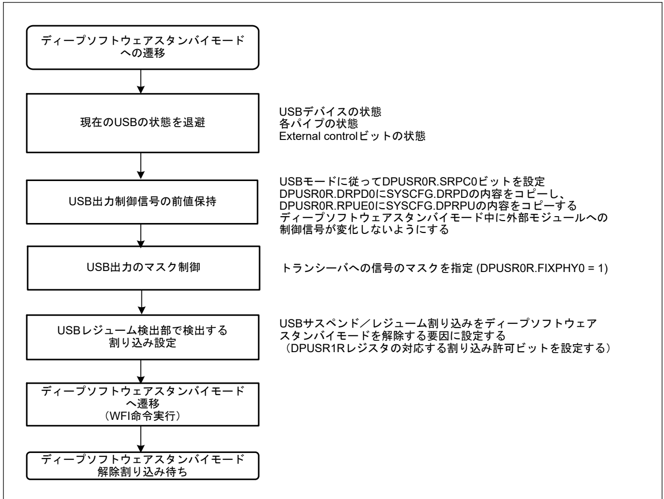
図 26.8 ホストコントローラ機能またはデバイスコントローラ機能選択時におけるディープソフトウェアスタンバイモード移行時の USBFS 設定フロー
