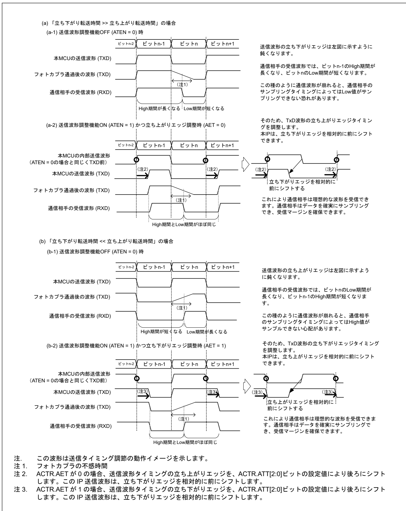
図 27.36 フォトカプラを通過する通信の送信動作の概要
