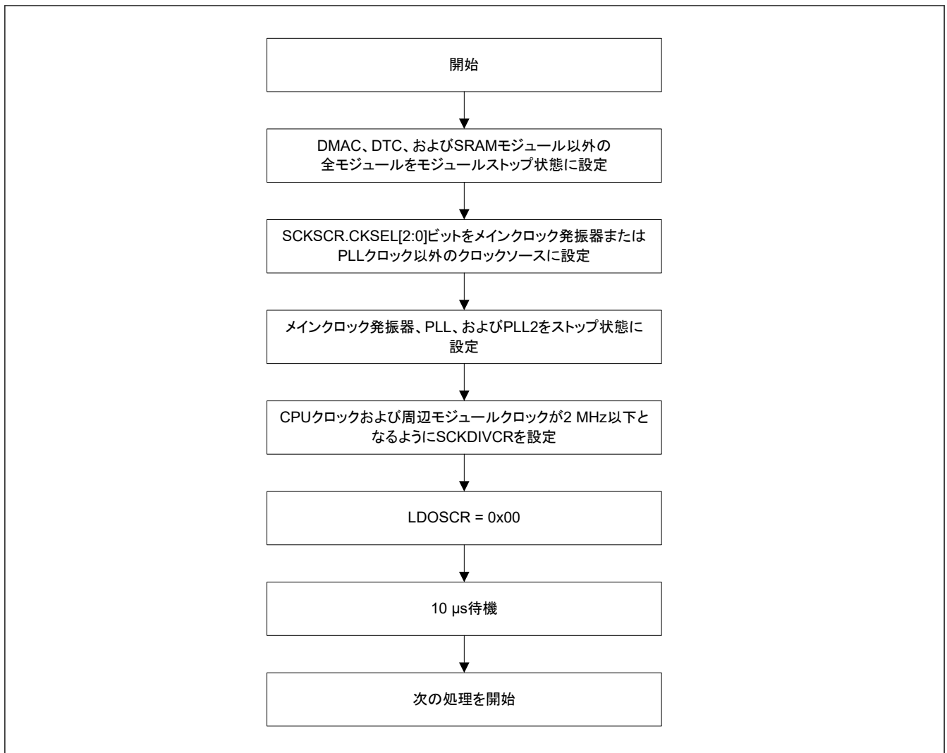
図 10.3 LDO0 および LDO1 のリスタートフロー
