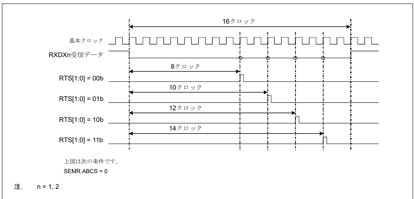
図 27.114 RXDXn 受信データサンプリングタイミング
