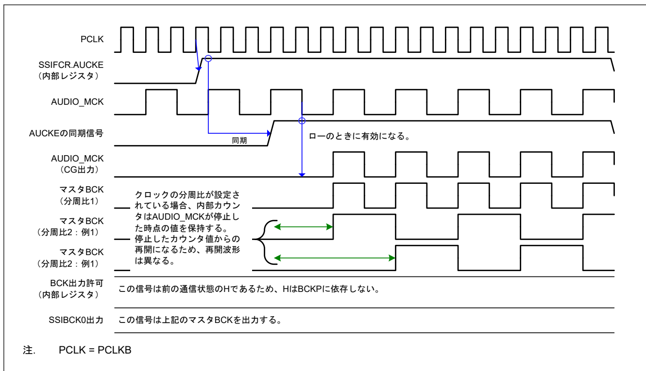
図 32.26 通信停止からマスタモード通信開始までの動作のタイミング図
