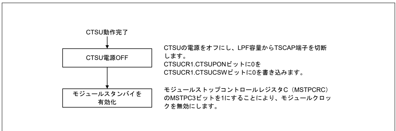
図 40.10 CTSU 停止フロー
