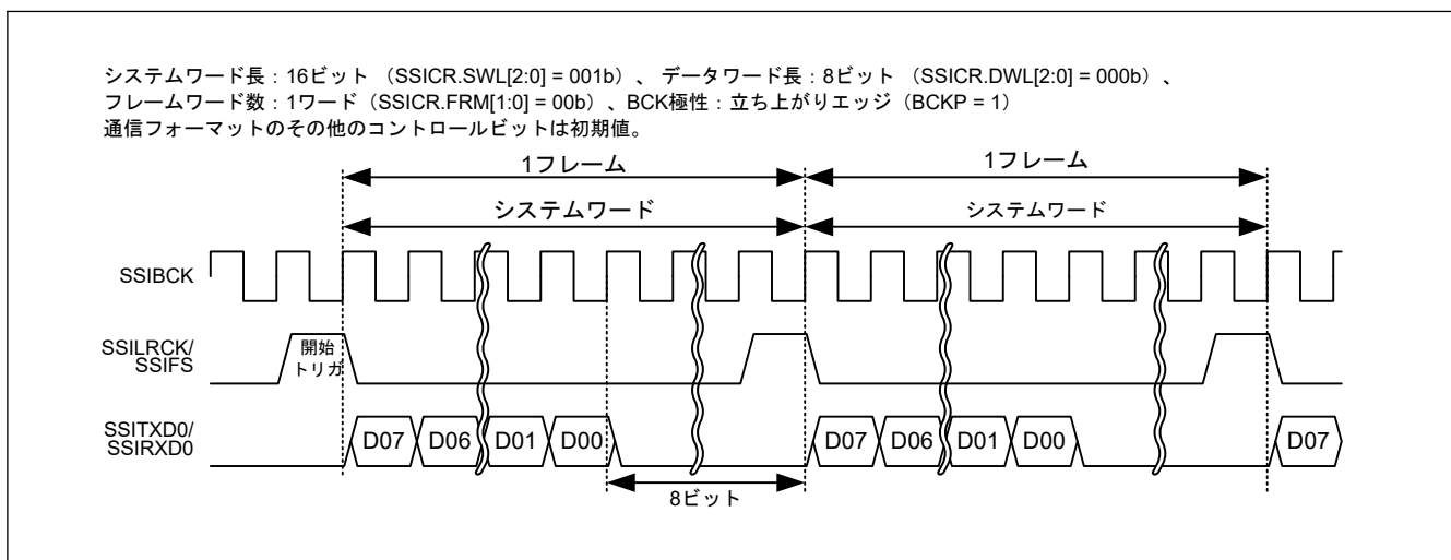
図 32.38 モノラルフォーマットにおけるショートフレーム (パディングあり、システムワード長 > データワード長)
