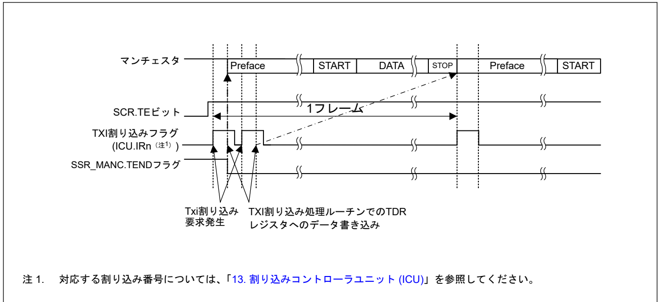
図 27.56 マンチェスタモードにおけるシリアル送信の送信開始動作の例 (プレフィスあり、CTS 機能なし)
