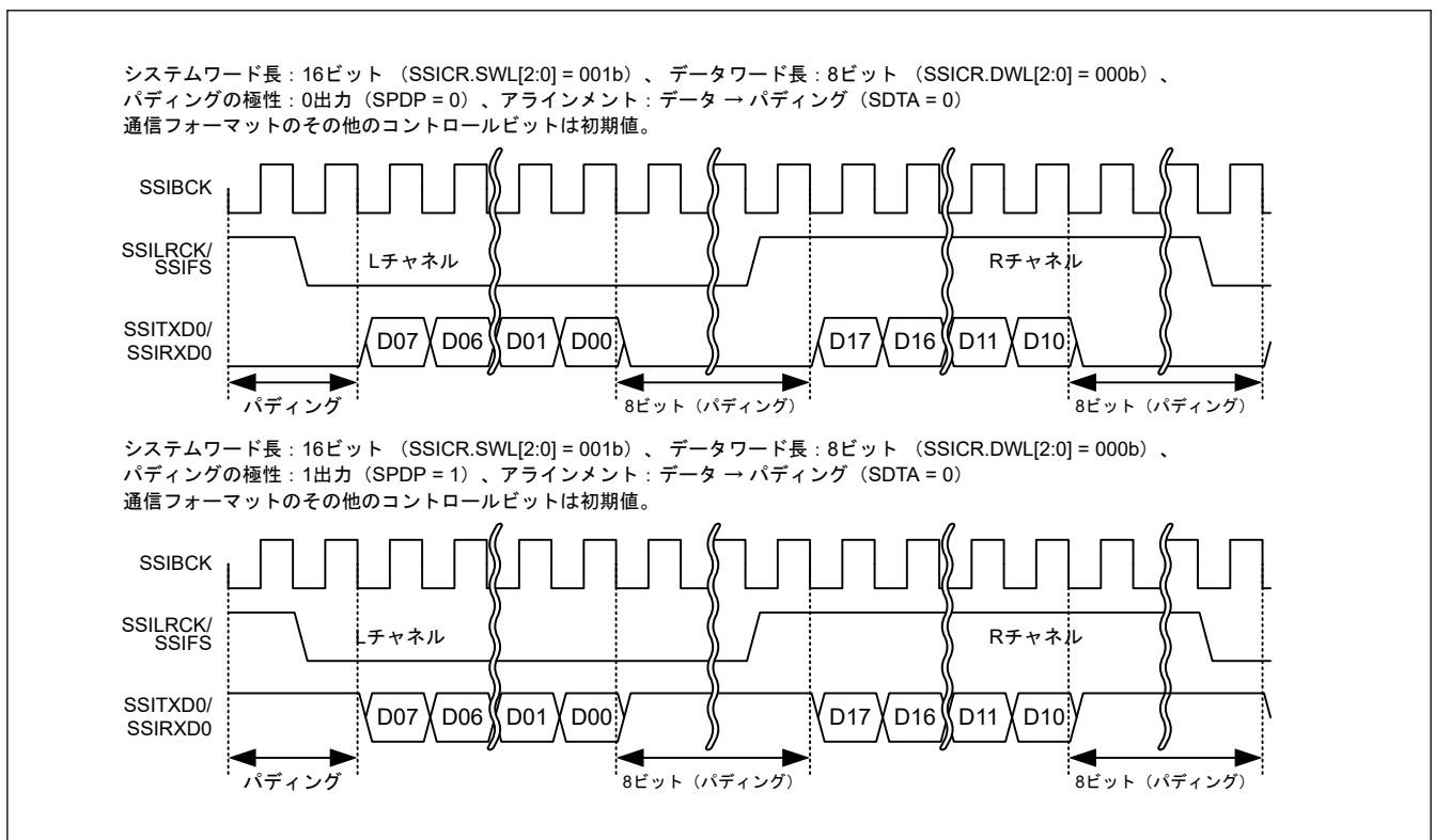
図 32.10 パディングビットの極性
