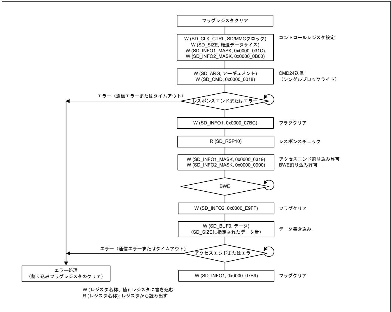
図 33.11 シングルブロックライト動作の例
