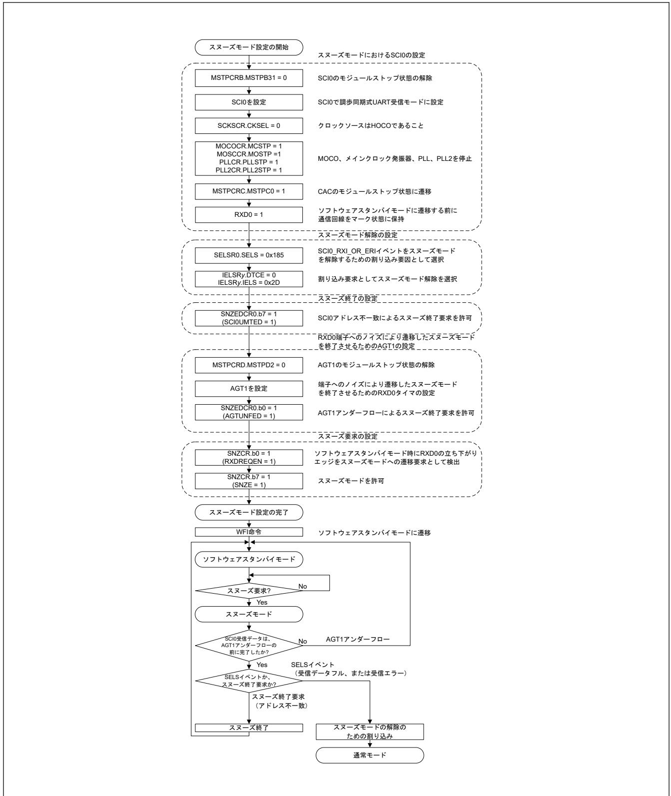
図 10.10 スリープモードエントリで SCI0 を使用するための設定例
