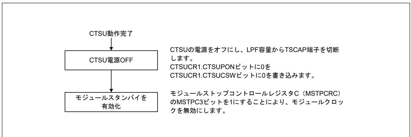
図 40.10 CTSUS 停止フロー
