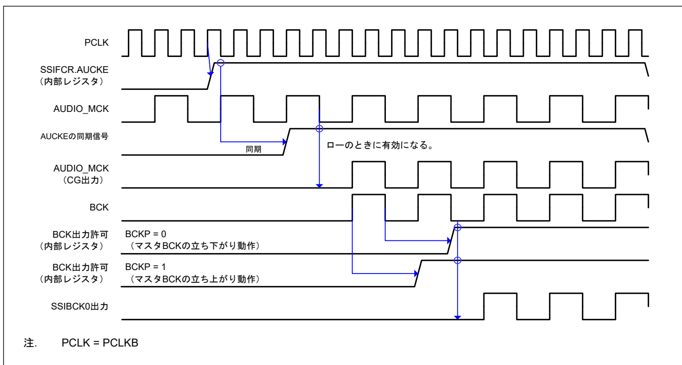
図 32.25 システムリセットからマスタモード通信開始までの動作のタイミング図
