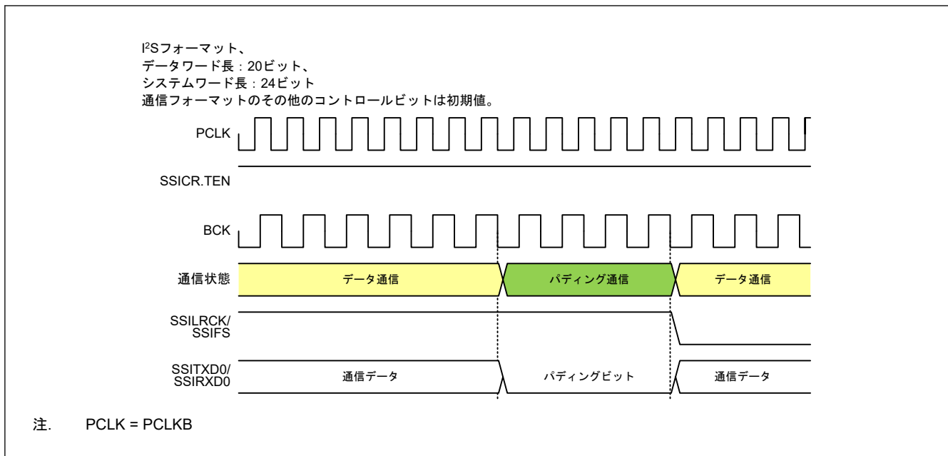
図 32.48 データ通信からパディング通信への遷移
