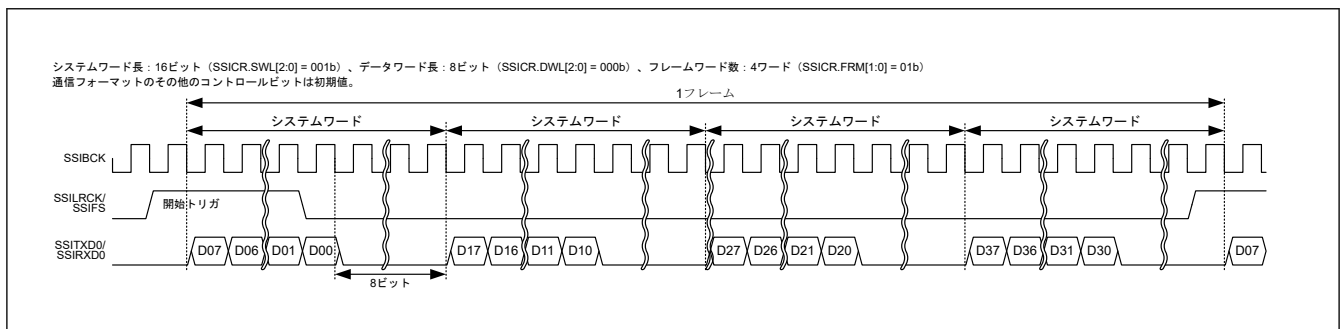
図 32.41 TDM フォーマット (パディングあり、システムワード長 > データワード長)
