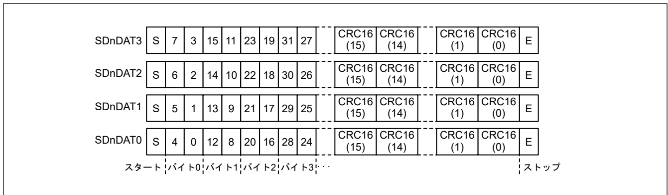
図 33.3 4 ビット幅モードの SDnDAT
