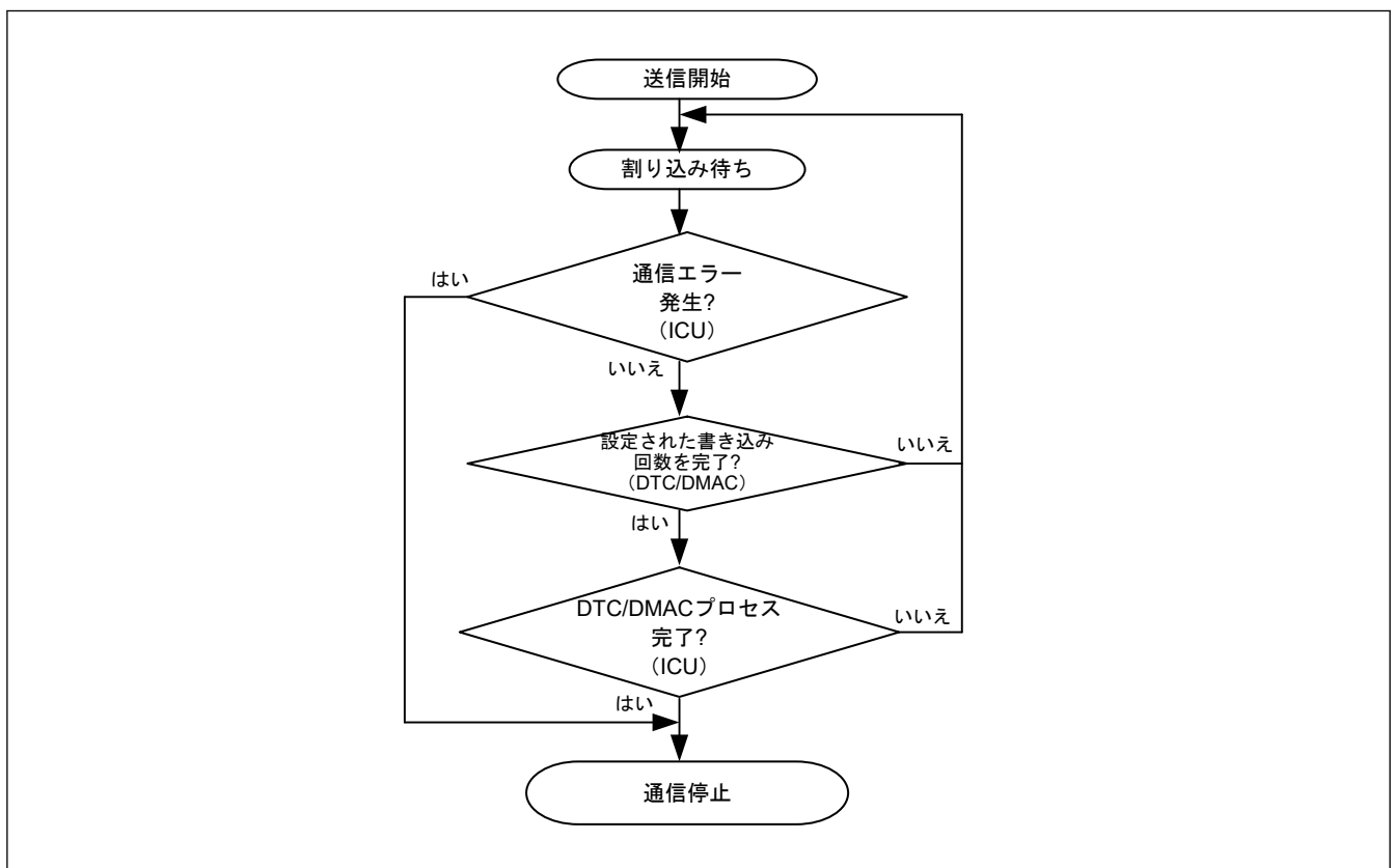
図 32.53 送信手順
