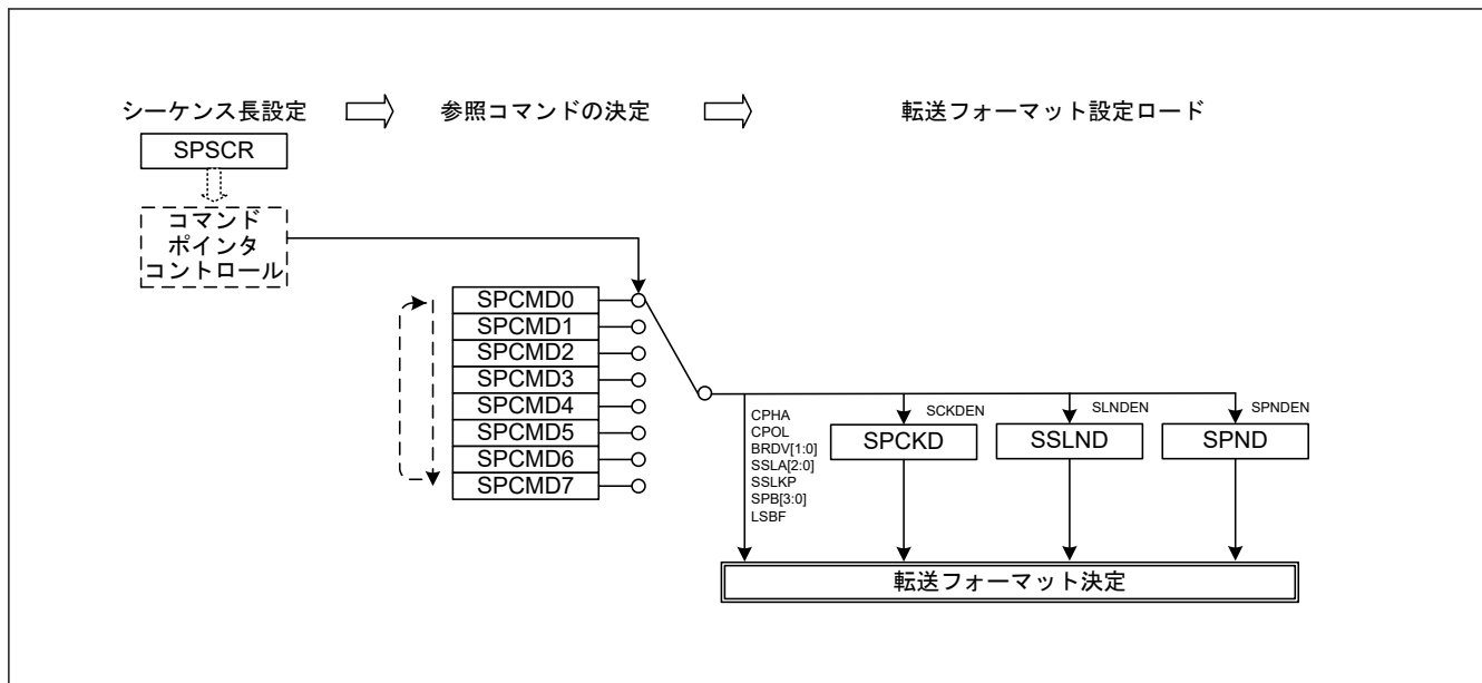
図 30.56 マスタモードでのシリアル転送方式の決定方法
