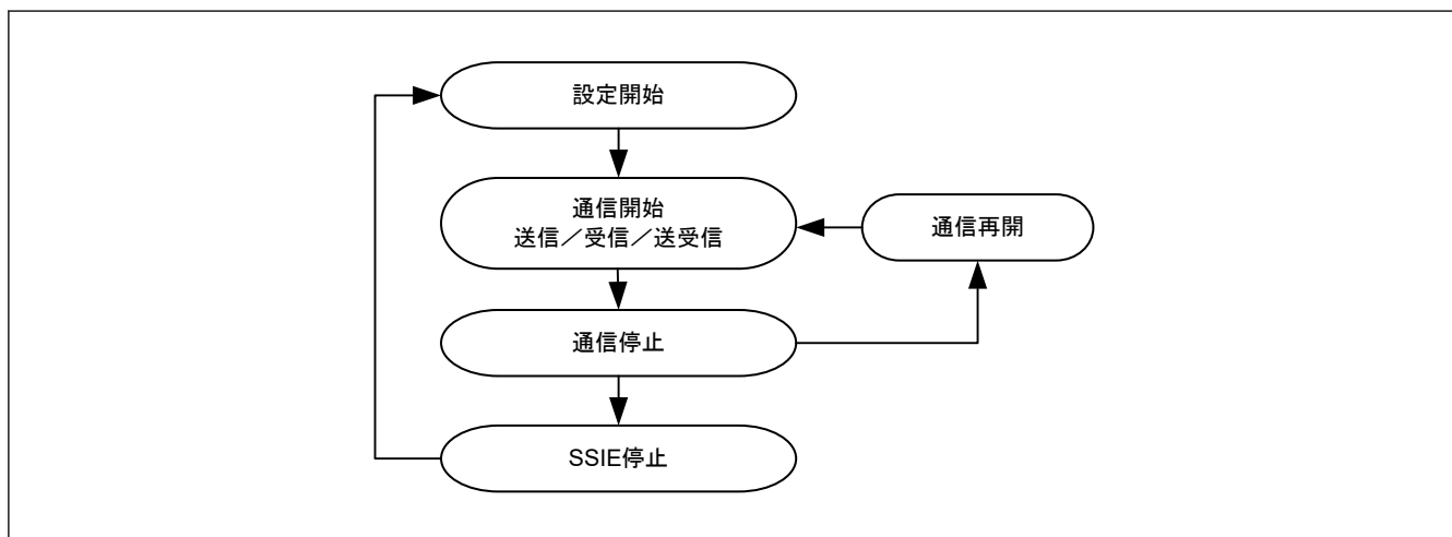
図 32.51 SSIE の通信動作
