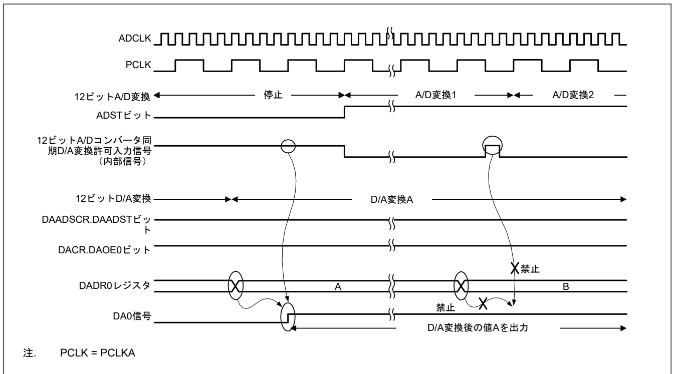
図 38.4 DAC12 が次からの同期 D/A 変換許可入力信号を取り込めない場合の例：ADC12
