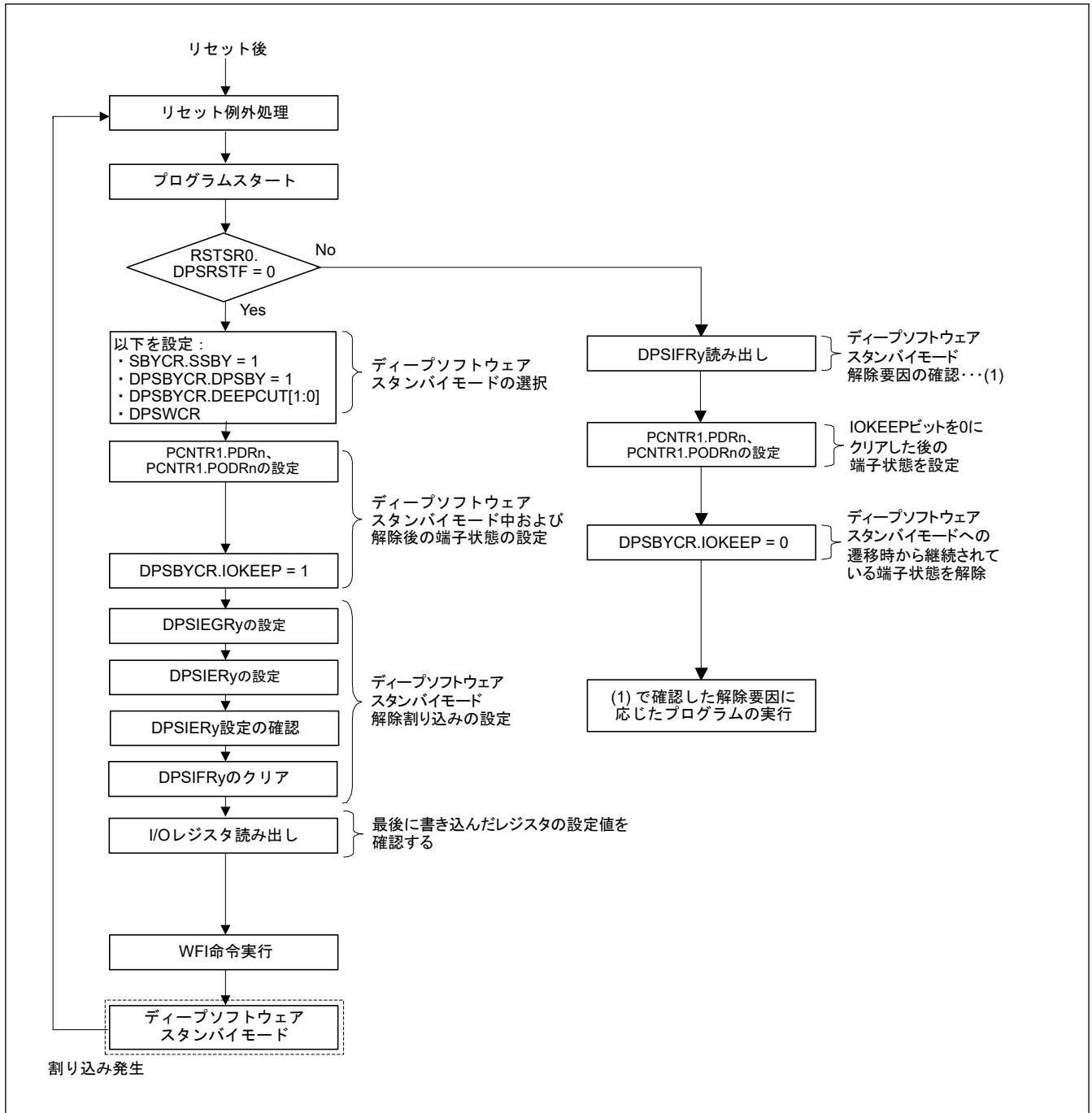
図 10.12 ディープソフトウェアスタンバイモード使用時のフローチャート例
