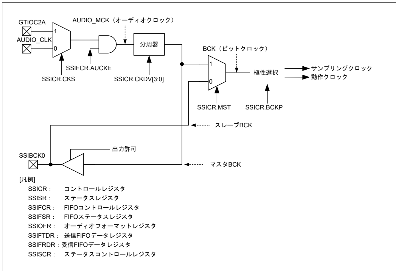
図 32.3 SSIE クロック構成
