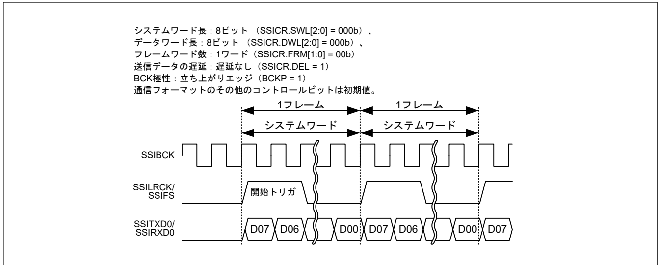
図 32.39 モノラルフォーマットにおけるロングフレーム (パディングなし)
