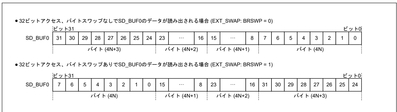
図 33.5 SD_BUF0 からの読み出し
