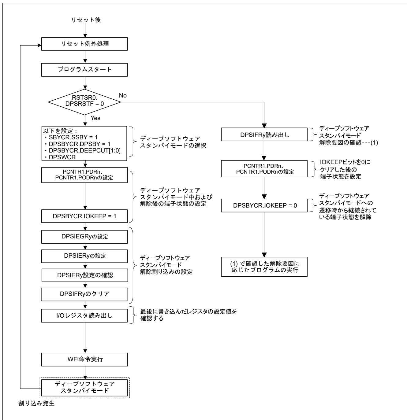
図 10.12 ディープソフトウェアスタンバイモード使用時のフローチャート例
