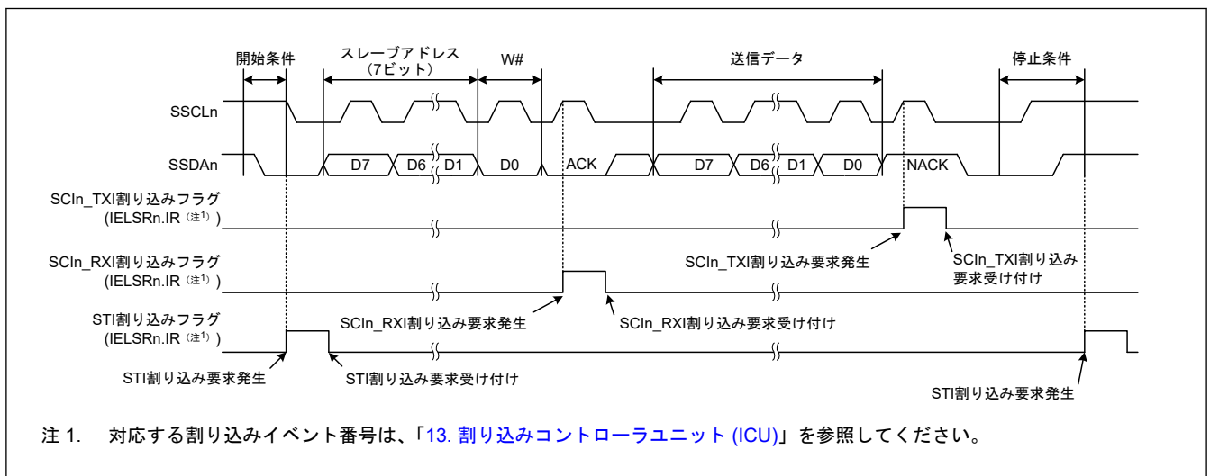
図 27.94 簡易 IIC モードにおけるマスタ送信の動作例 2 (7 ビットスレーブアドレス、ACK 割り込み、NACK 割り込み使用時)
