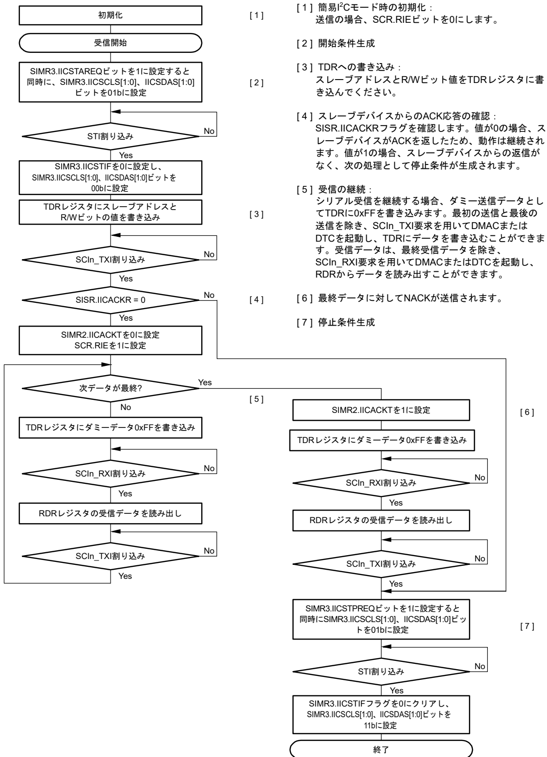
図 27.97 簡易 IIC モードにおけるマスタ受信のフローチャート例 (送信割り込み、受信割り込み使用時)
