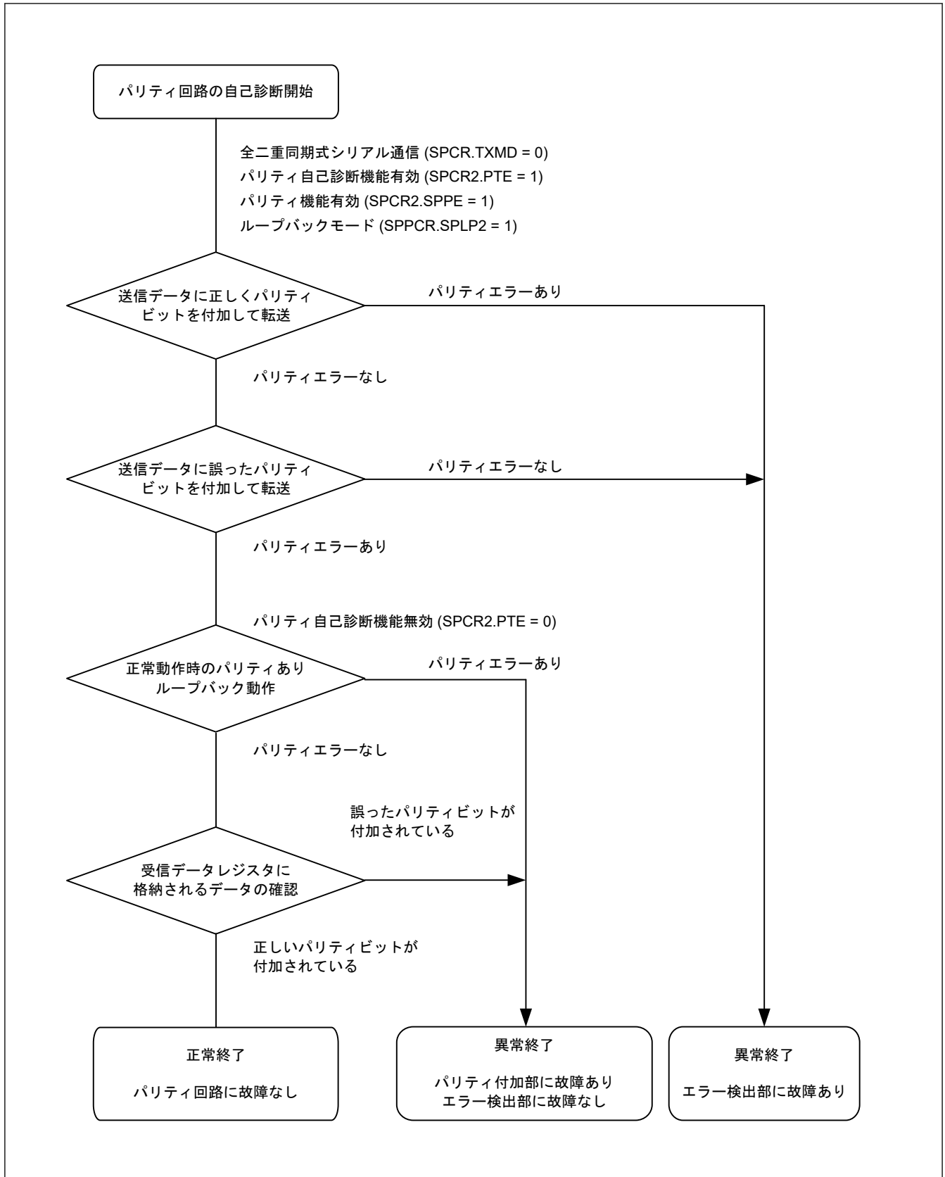
図 30.62 パリティ回路の自己診断フロー
