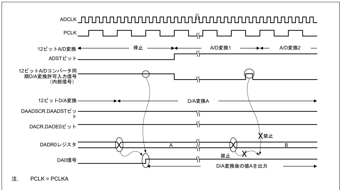
図 38.4 DAC12 が次からの同期 D/A 変換許可入力信号を取り込めない場合の例：ADC12 (ユニット 1)
