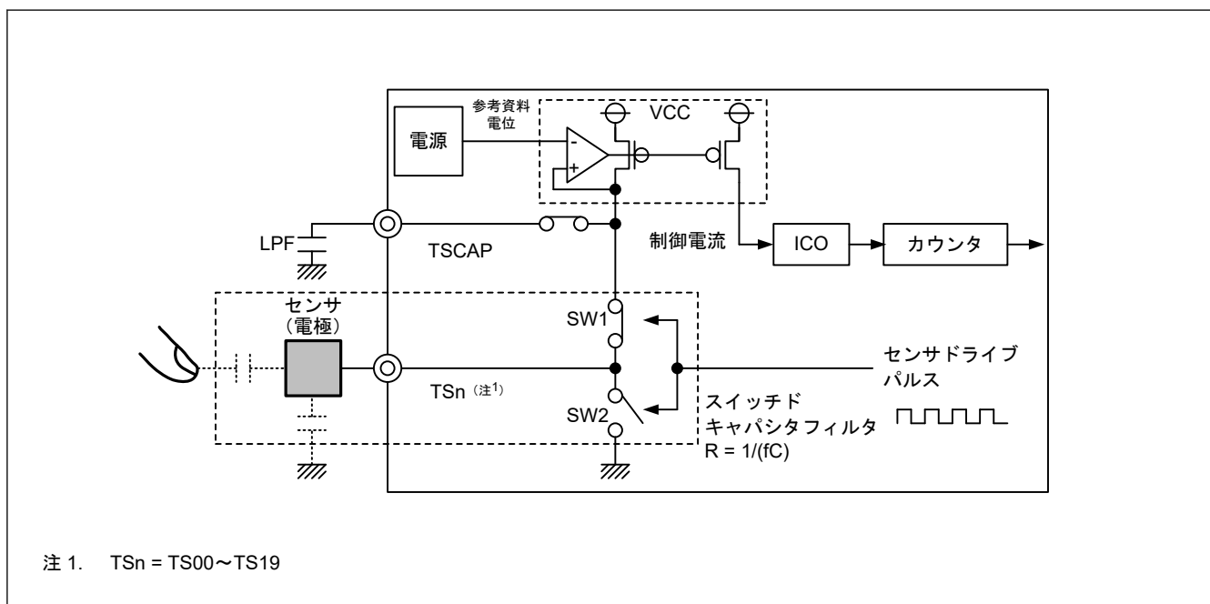
図 40.4 計測部回路
