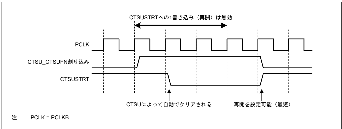
図 40.21 再開時の注意事項
