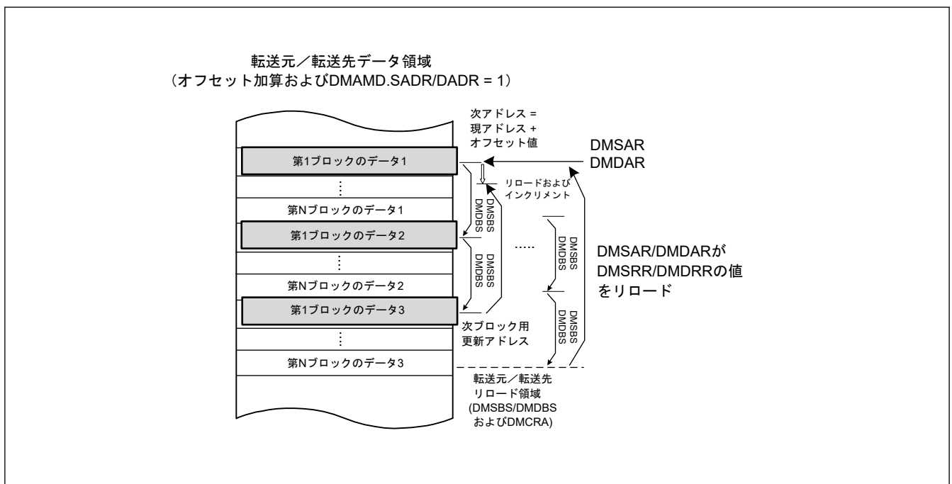
図 16.17 オフセット加算モードにおけるアドレス更新 (DMAMD.SADR = 1 かつ DMAMD.DADR = 1 の場合)
