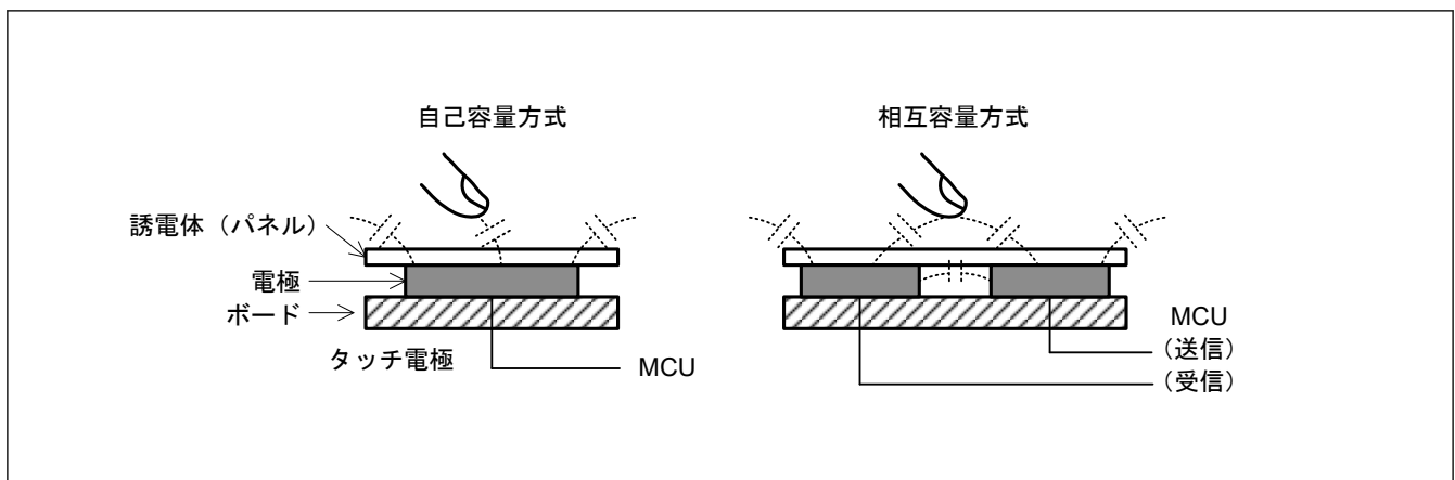
図 40.2 自己容量方式と相互容量方式
