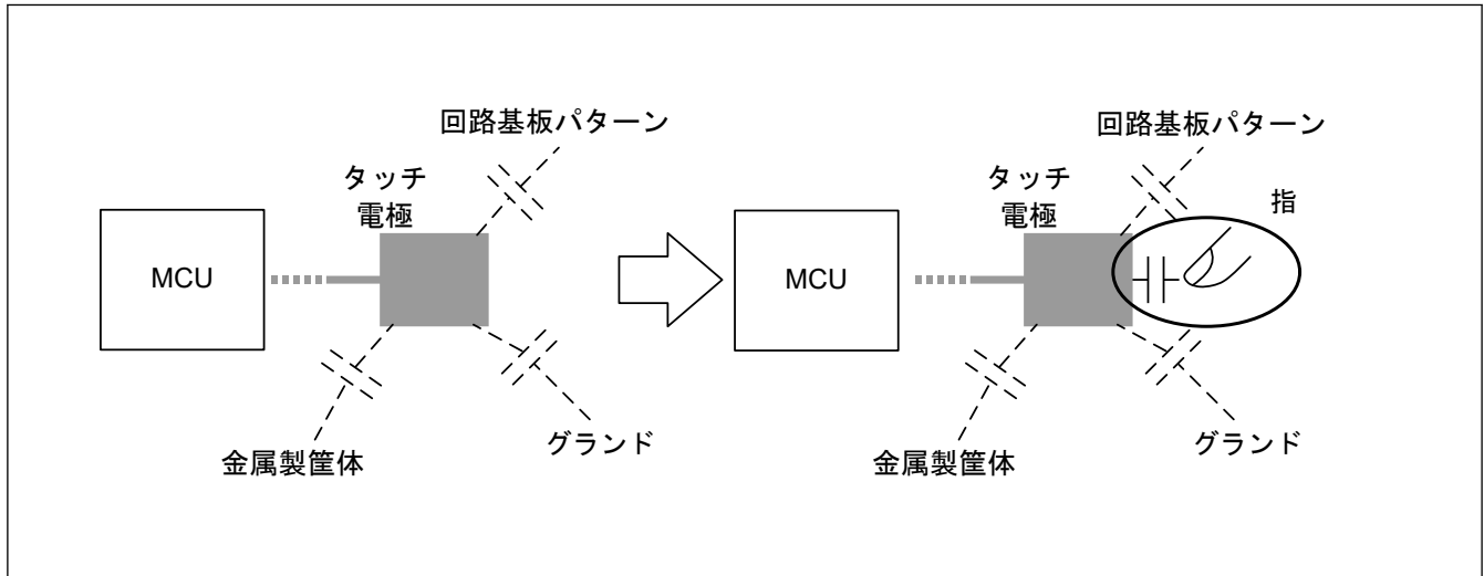
図 40.1 指による静電容量の増加
