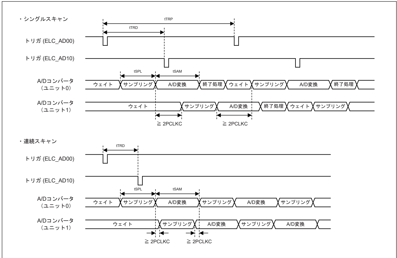
図 37.24 インターリーブ動作におけるトリガ入力タイミング
