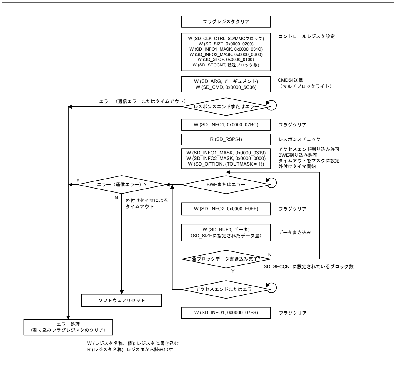
図 33.15 外付けタイマによるマルチブロックライト動作の例
