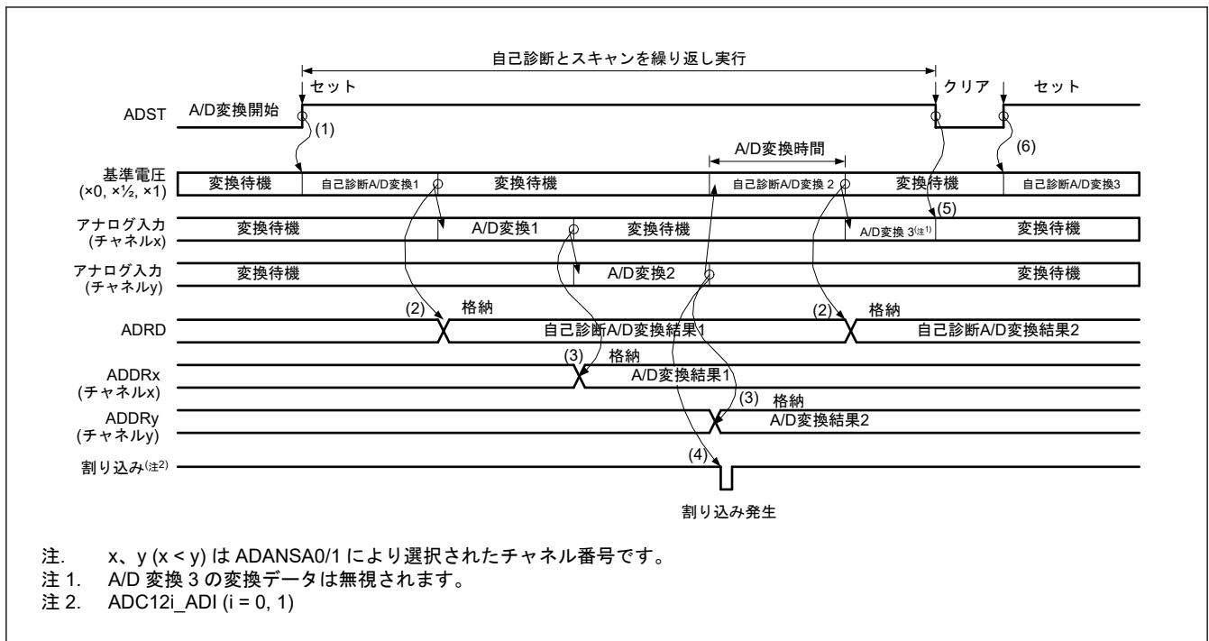
図 37.14 連続スキャンモードの基本動作例 (アナログ入力 (チャンネル x, y) 選択+自己診断)
