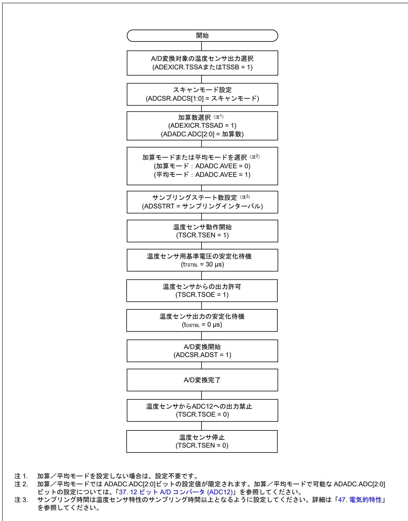
図 39.2 TSN の使用手順例
