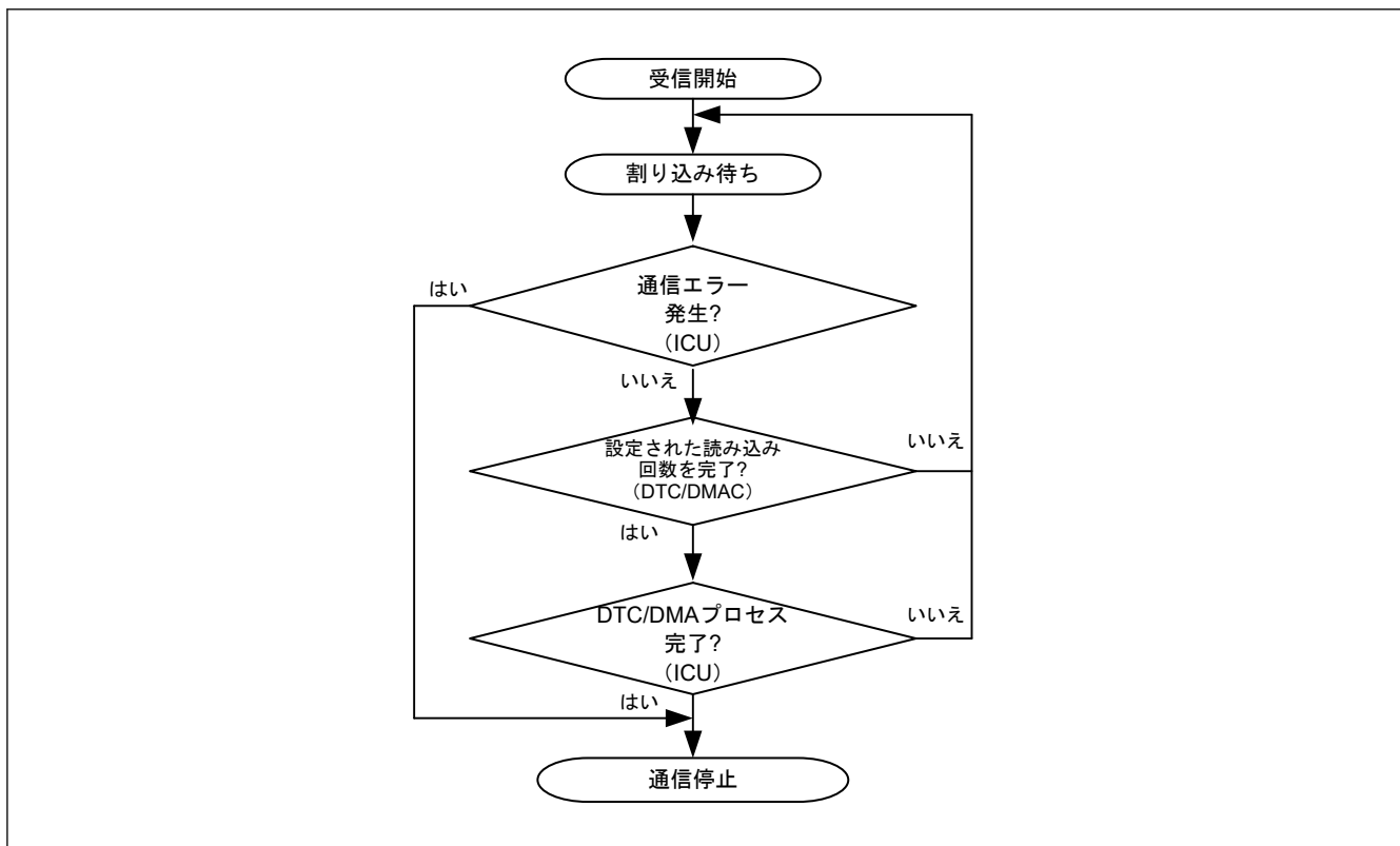
図 32.55 受信手順
