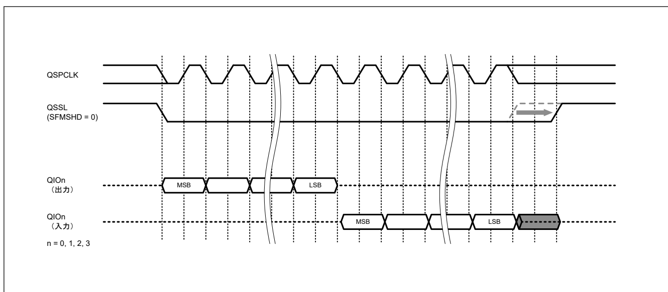
図 31.12 SFMSHD ビットを使用した QSSL 信号のホールド時間調整
