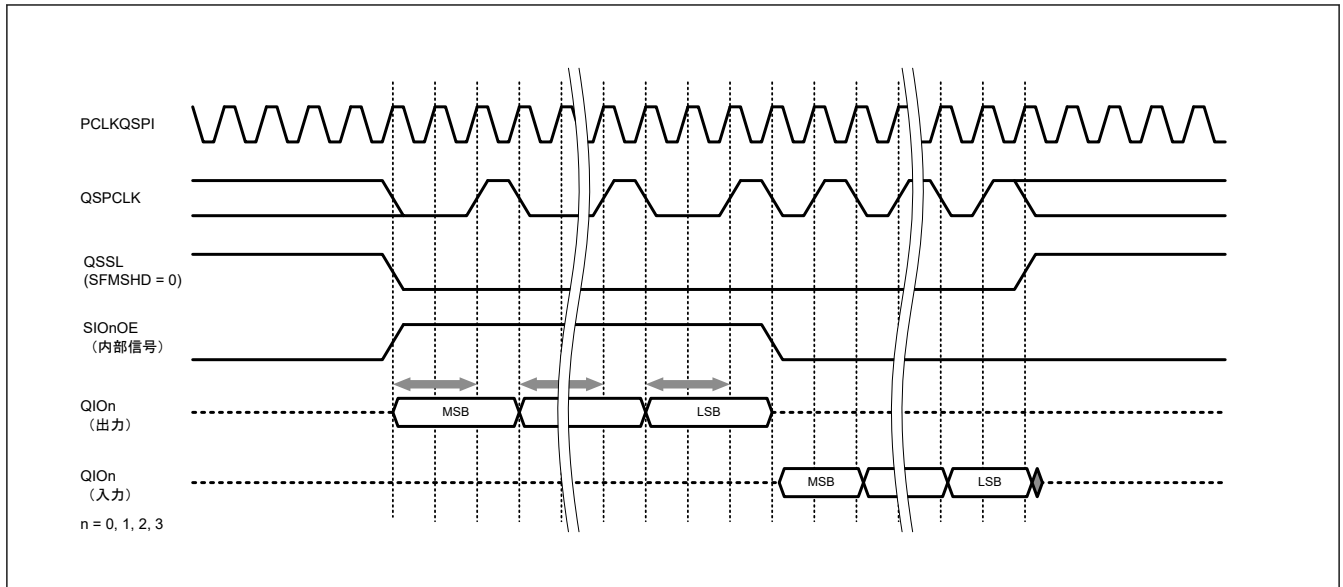
図 33.15 SFMOSW ビットを使用したシリアルデータ出力のセットアップ時間調整
