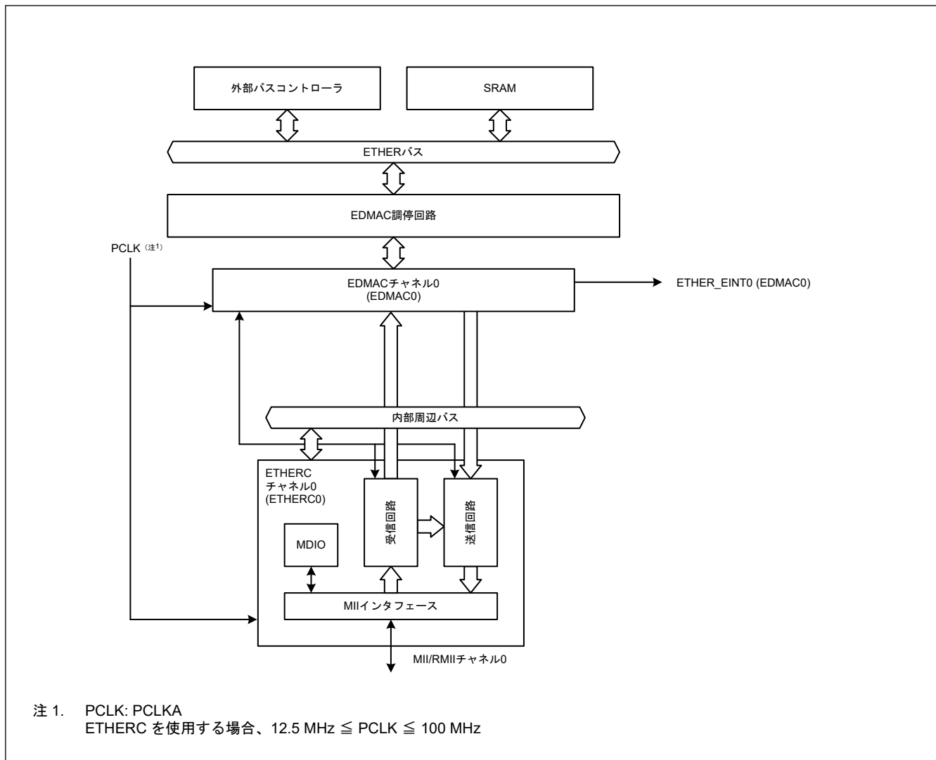
図 26.1 ETHERC 構成
