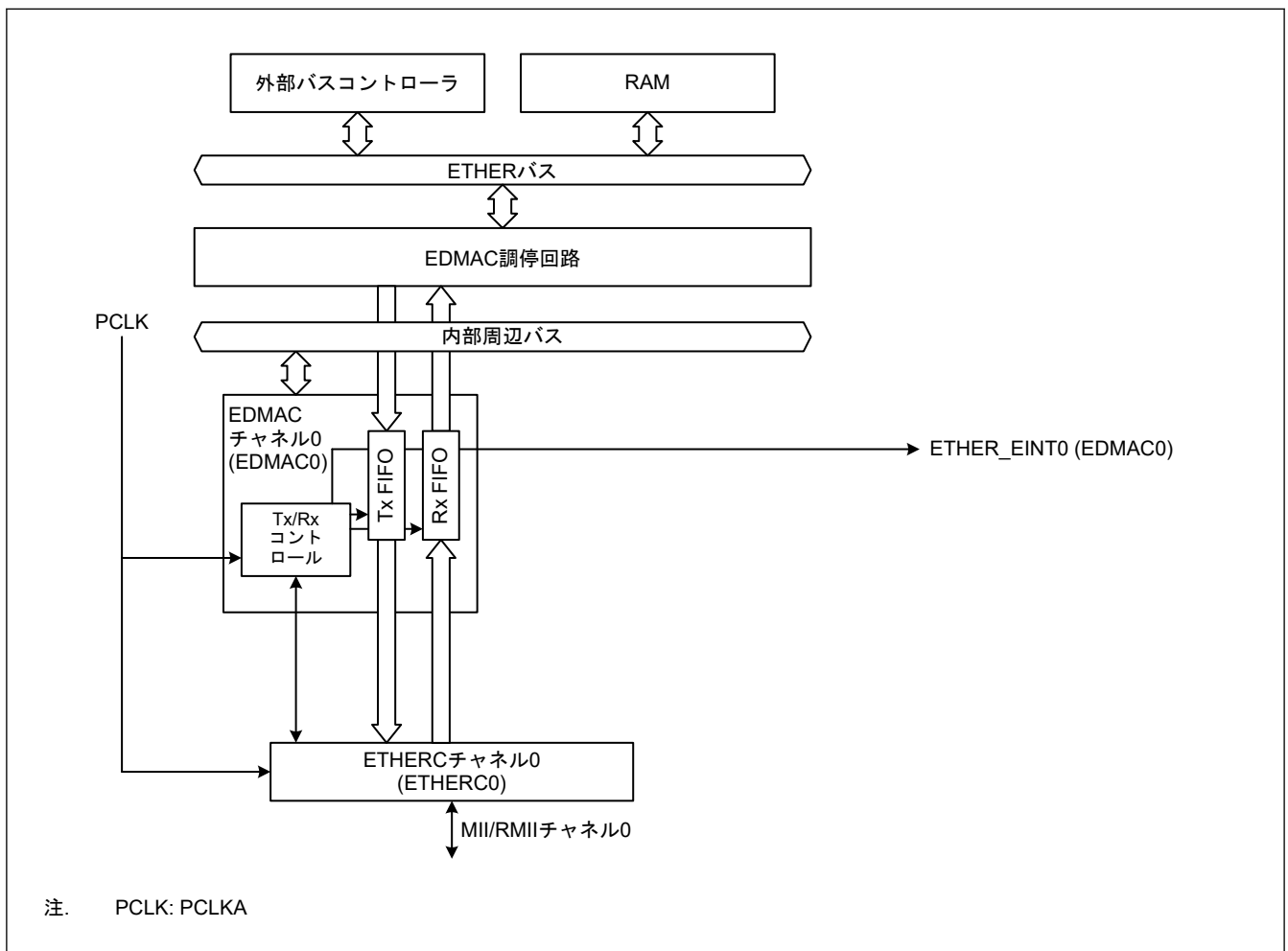
図 27.1 EDMAC の構成
