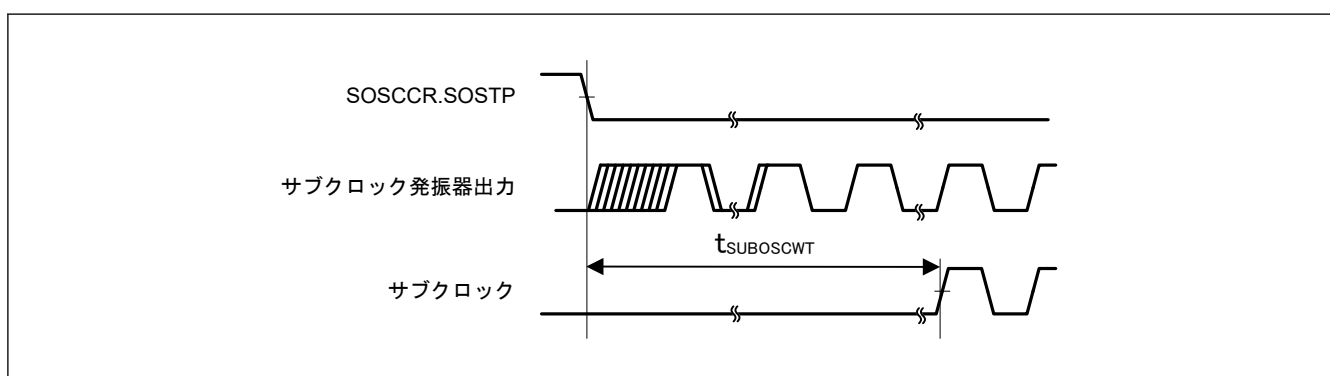
図 50.12 サブクロック発振開始タイミング
