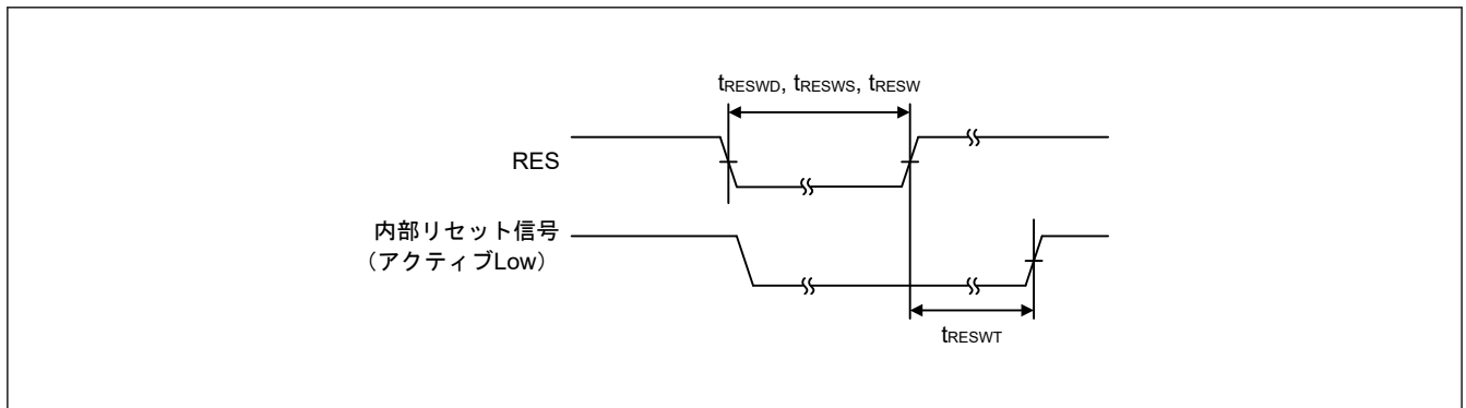
図 50.14 リセット入カタイミング
