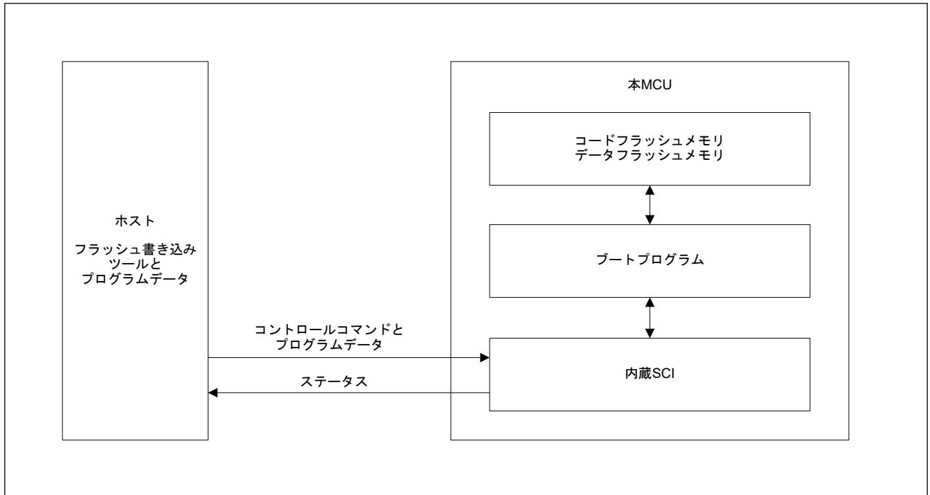
図 47.43 ブートモード (SCI インタフェース) 時のシステム構成
