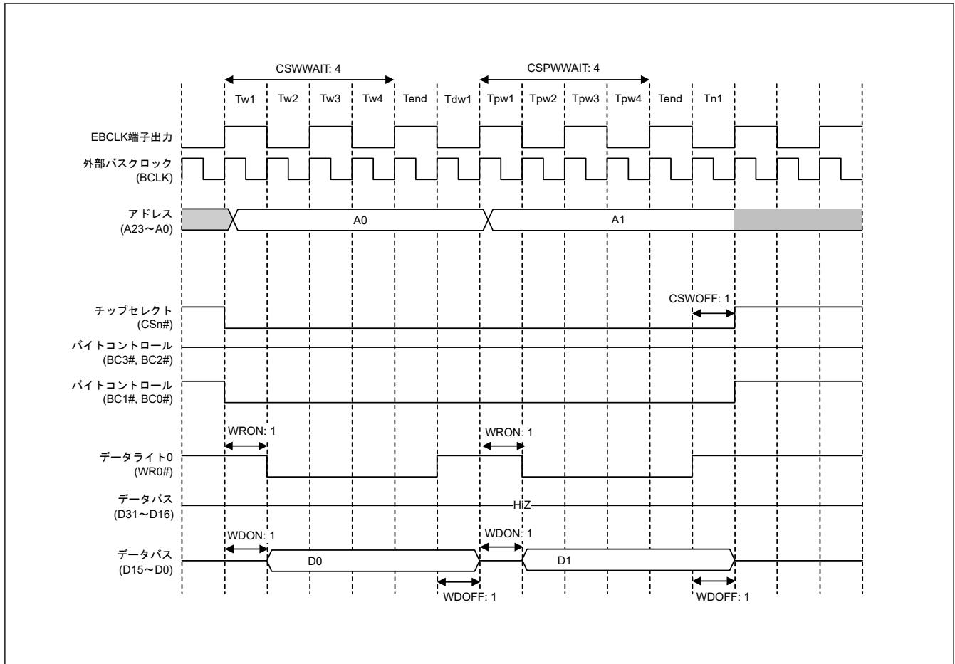
図 14.22 ページライトアクセスの動作例 (EBCLK 端子出力選択ビットで BCLK の 2 分周を設定した場合、および 1 転送要求に対して 2 回バスアクセスが発生する場合、1 ライトストロブモード時) (n = 0~7)
