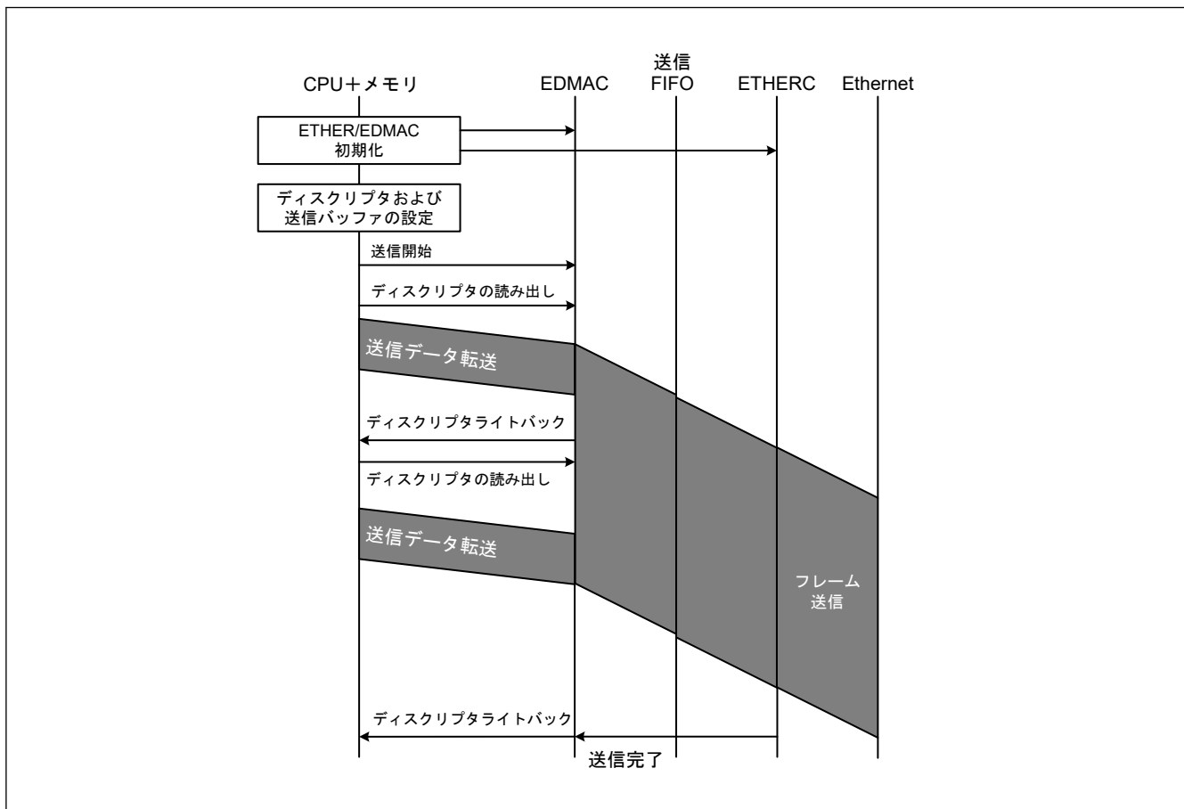
図 27.5 送信フローの例
