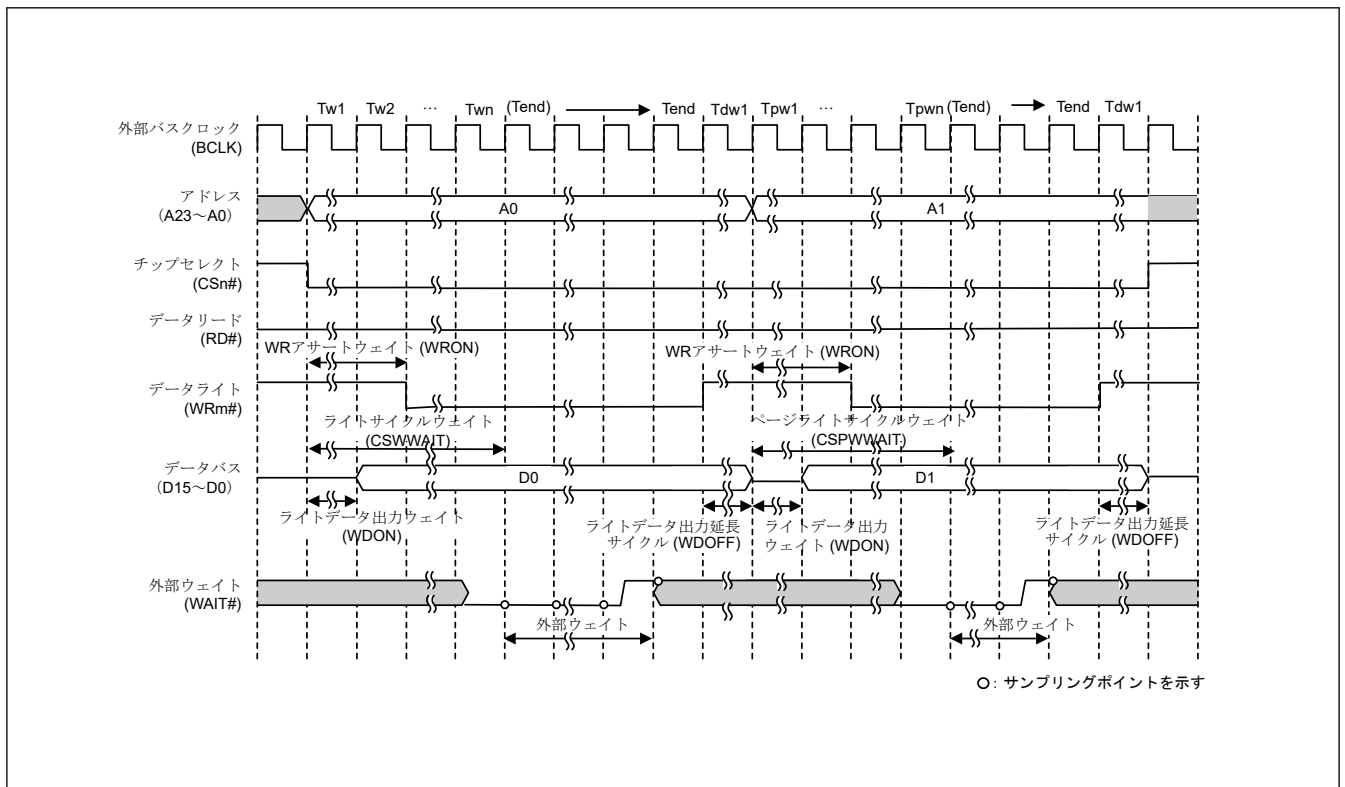
図 14.28 バイトストローブモード時の 16 ビットバス空間に対するページライトアクセスの外部ウェイトタイミング例 (EBCLK 端子出力選択ビットで BCLK の 1 分周を選択した場合) (n = 0~7、m = 0、1)
