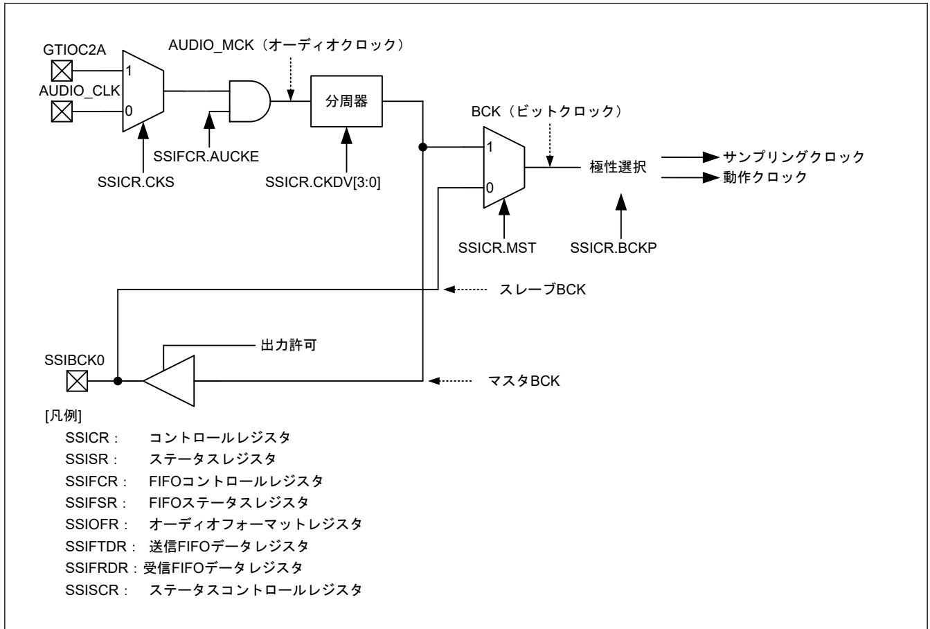
図 35.4 SSIE クロック構成
