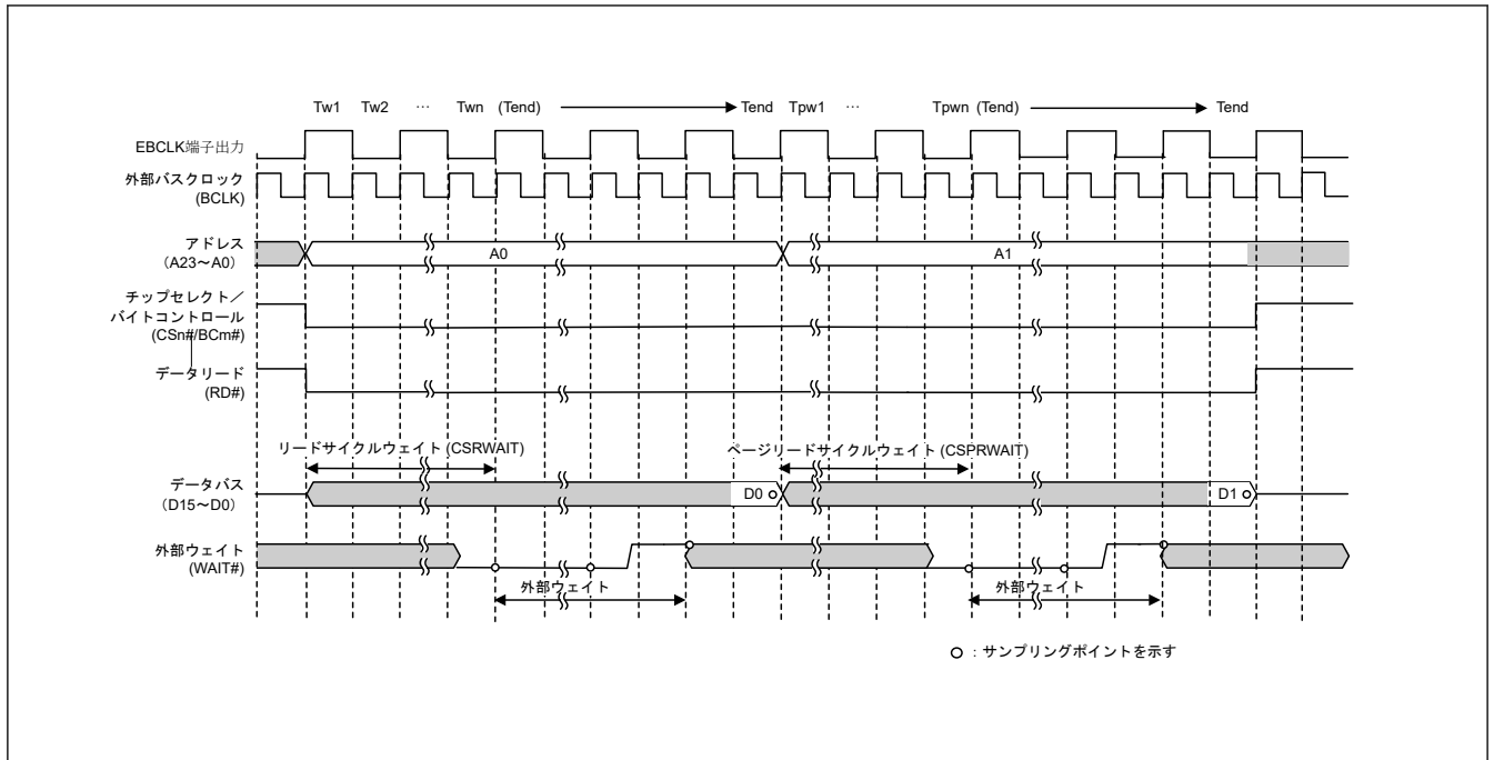
図 14.27 16 ビットバス空間に対するページリードアクセスの外部ウェイトタイミング例 (EBCLK 端子出力選択ビットで BCLK の 2 分周を選択した場合) (n = 0~7、m = 0、1)
