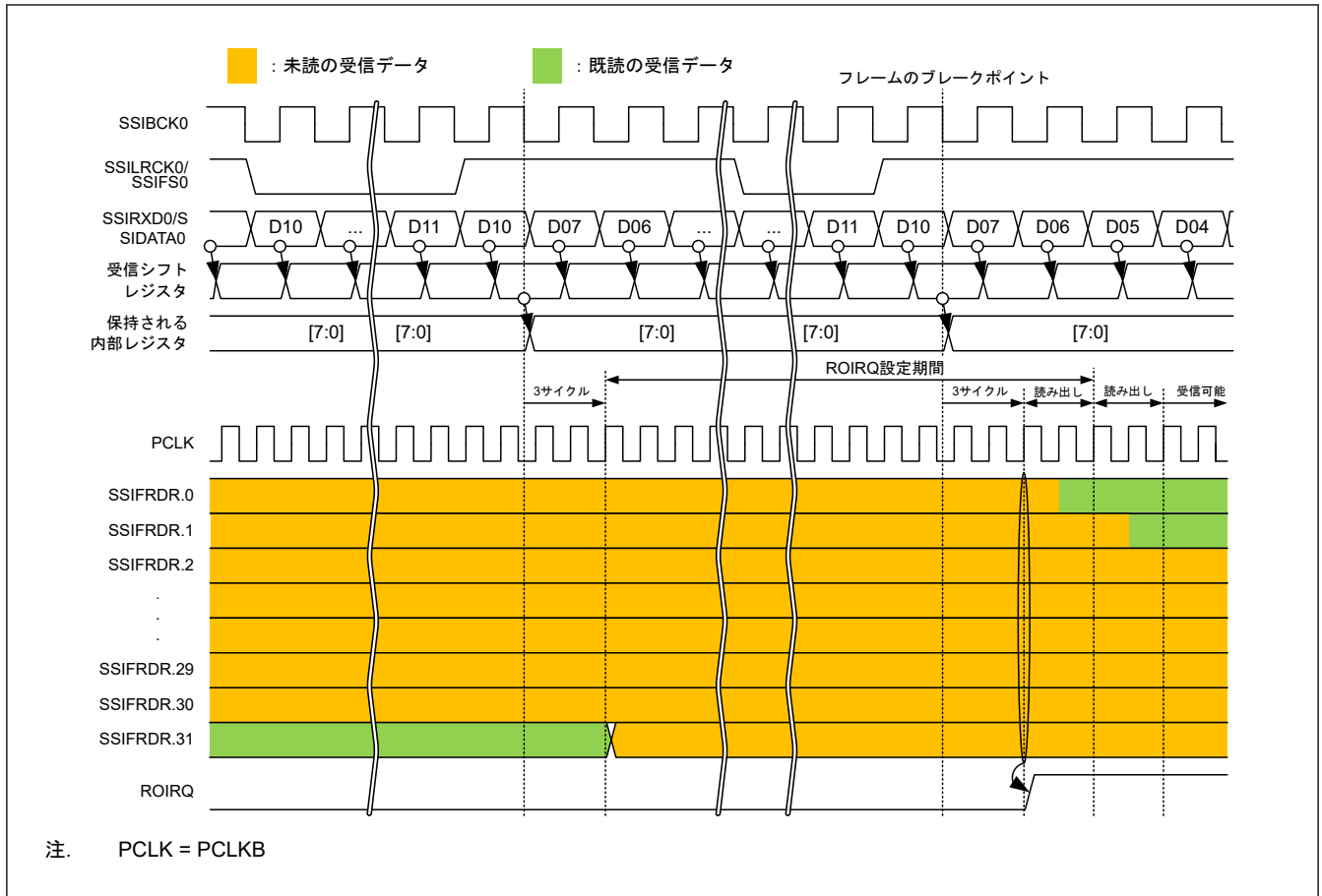
図 35.16 ROIRQ 設定タイミング
