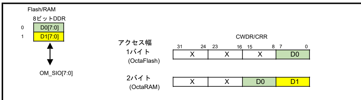
図 34.12 OctaFlash および OctaRAM スペースの構成レジスタデータアラインメント
