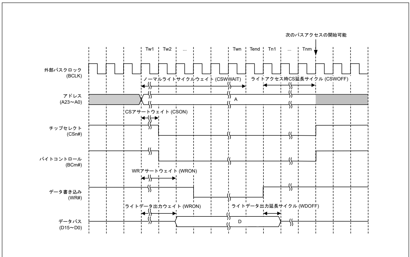
図 14.8 ノーマルライトアクセスのバスタイミング（1 ライトストロブモード）（n = 0~7、m = 0~1）
