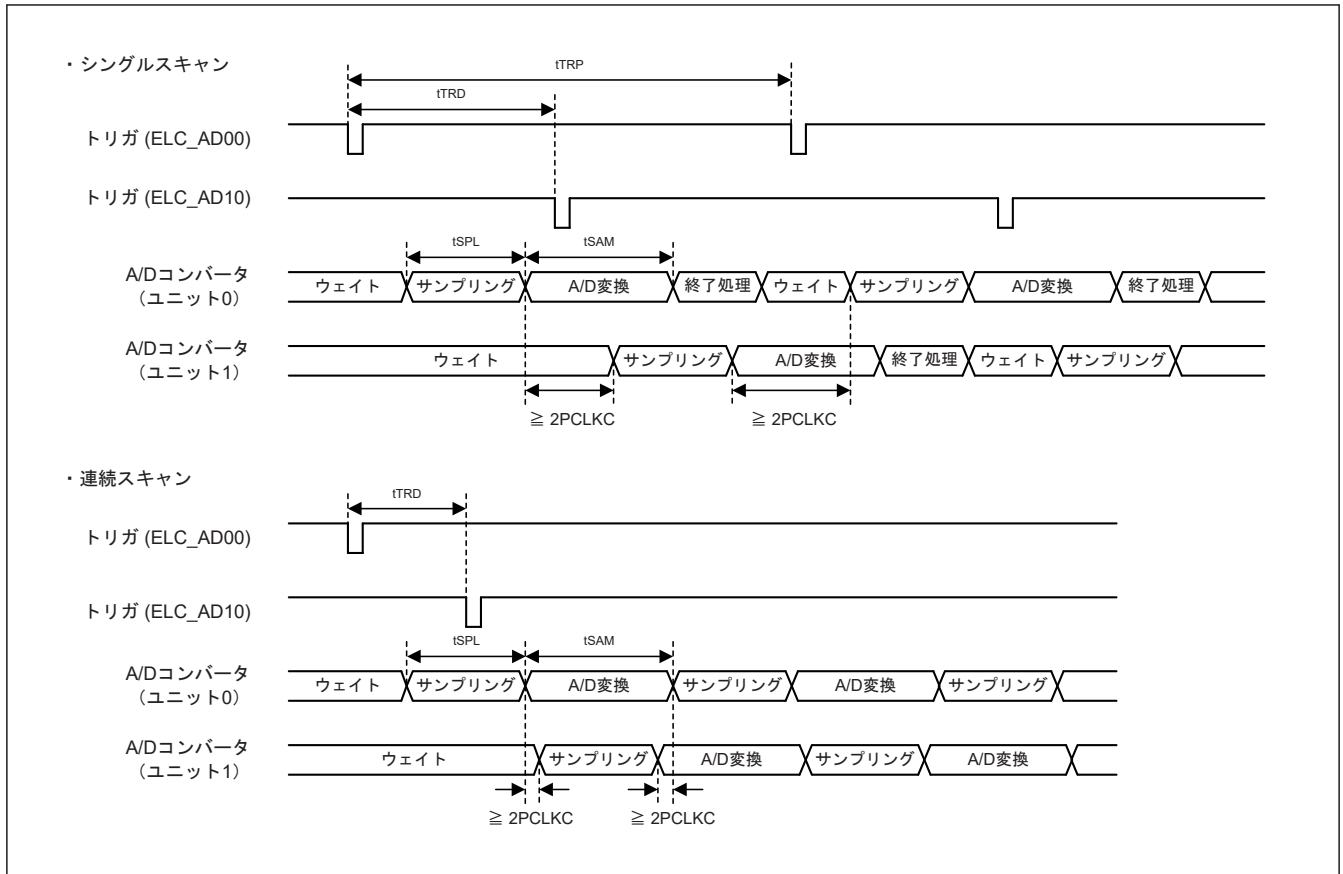
図 40.24 インターリーブ動作におけるトリガ入力タイミング
