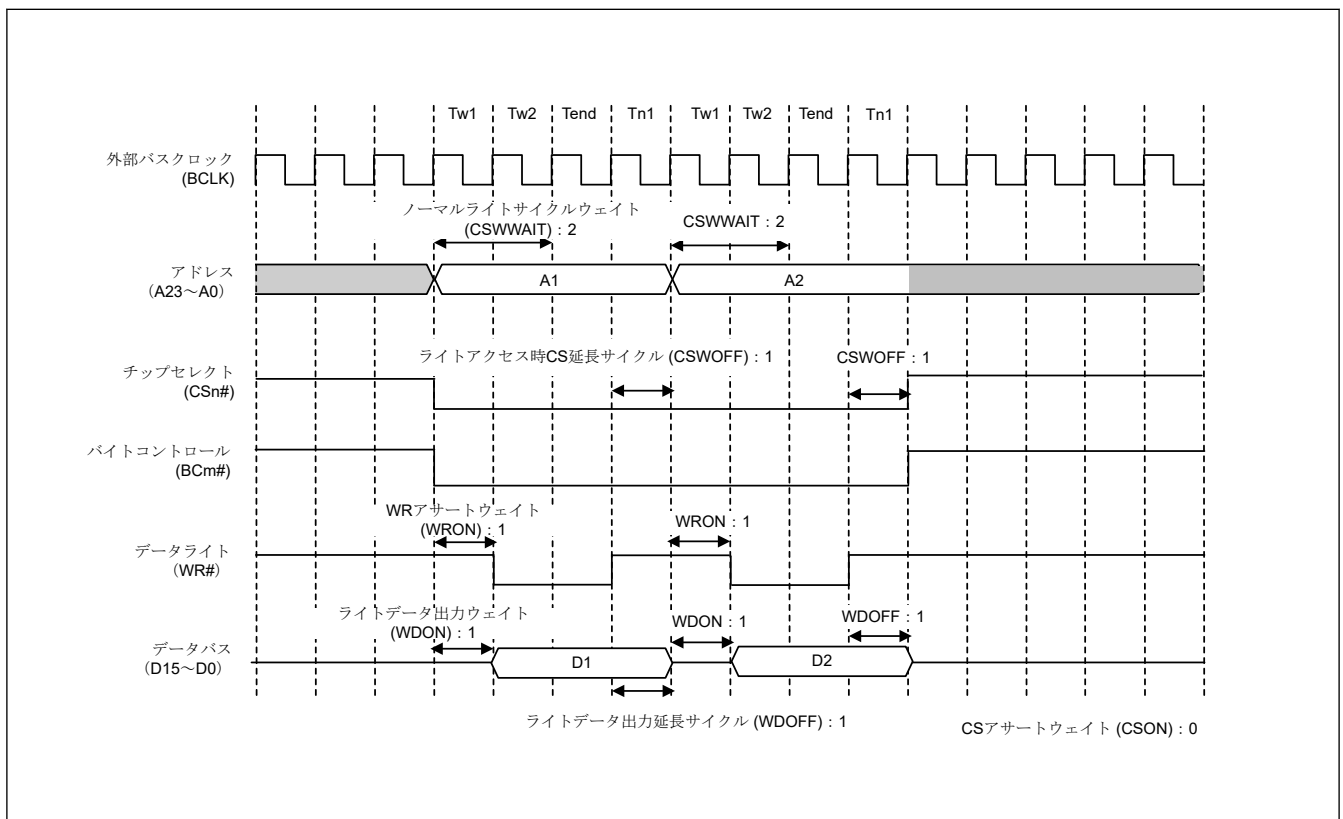
図 14.11 ノーマルライトアクセスの動作例 (1 転送要求に対して 2 回バスアクセスが発生する場合、1 ライトストロブモード時) (n = 0~7、m = 0~1)
