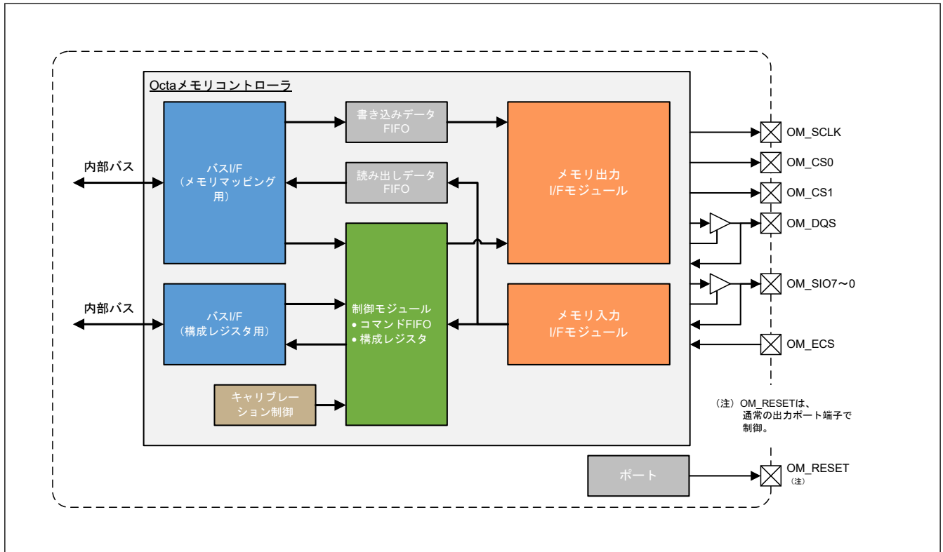
図 34.1 ブロック図
