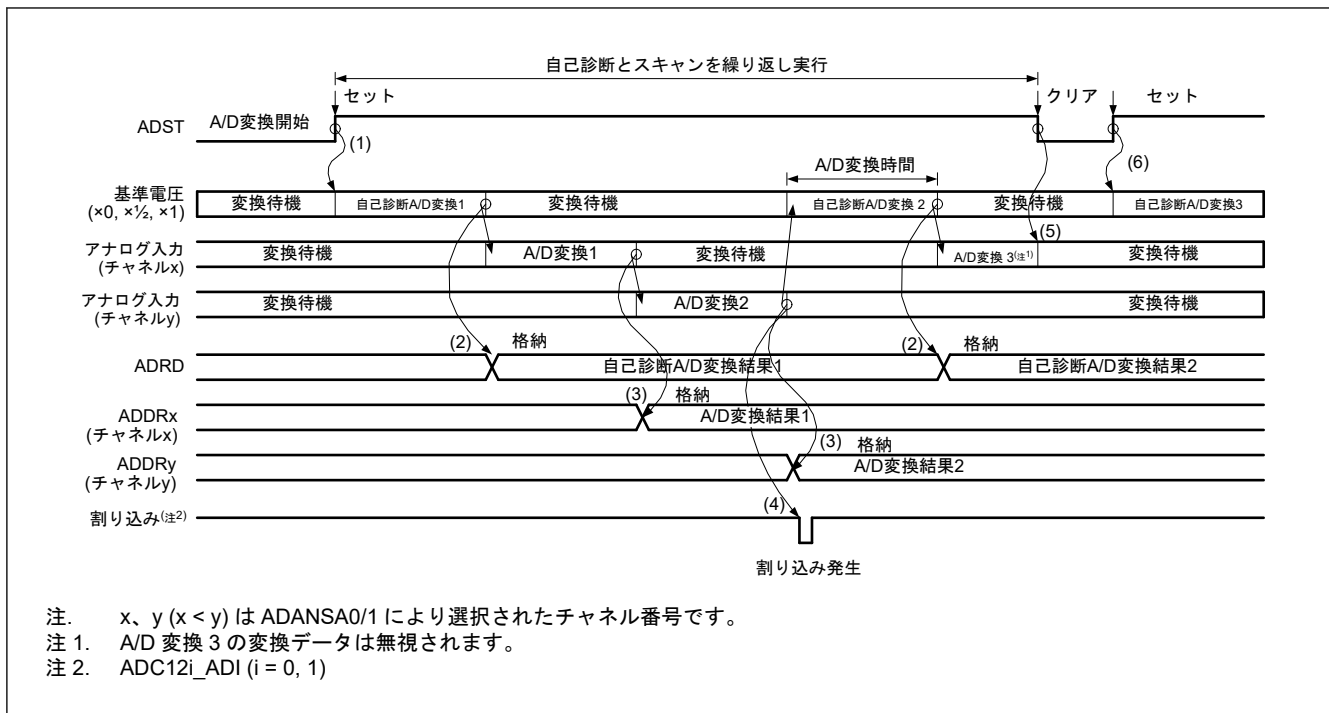
図 40.14 連続スキャンモードの基本動作例 (アナログ入力 (チャンネル x、y) 選択+自己診断)
