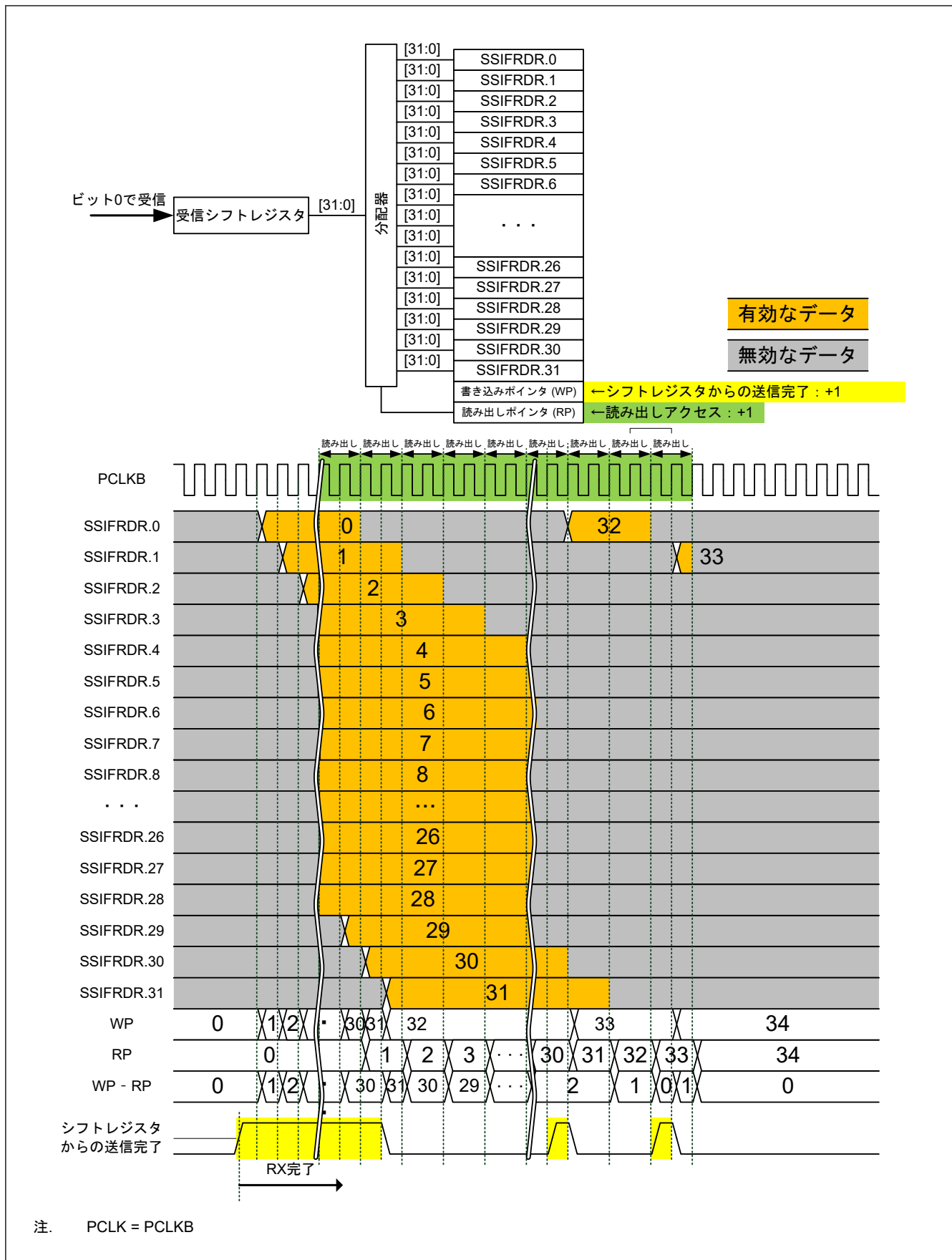
図 35.32 受信 FIFO データレジスタと受信シフトレジスタの構成、および FIFO の動作例
