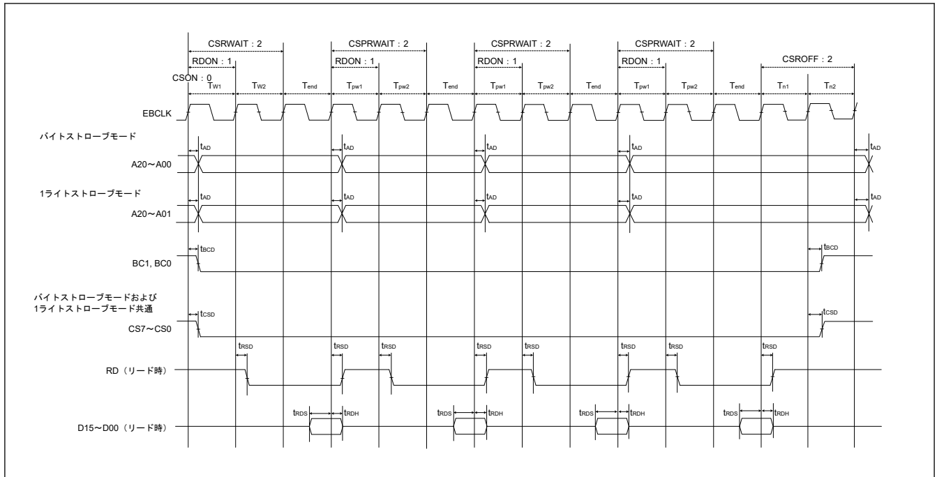
図 50.24 バスクロック同期を使用したページリードサイクルの外部バスタイミング
