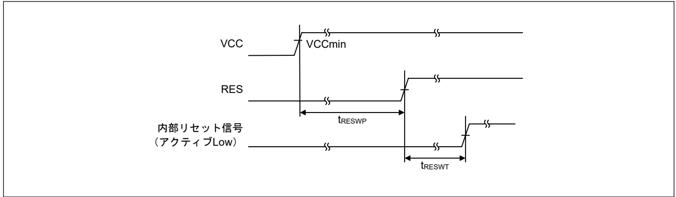
図 50.13 VCC が V POR 電圧しきい値を超える条件下での RES 端子入カタイミング
