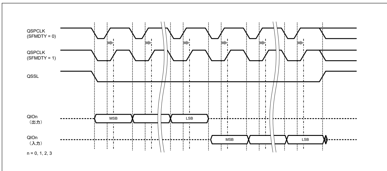
図 33.10 PCLKA を 3 通り倍した場合の SFMDTY ビットを使用した QSPCLK 信号デューティー比補正例
