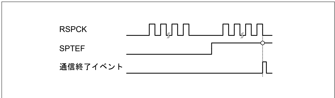
図 32.64 通信終了イベント出力タイミング (送信スレーブモード、クロック同期式動作)
