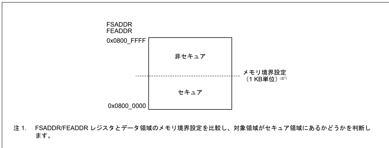
図 47.37 データ領域のセキュア/非セキュア領域
