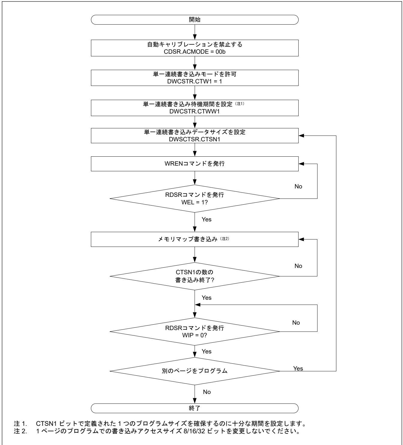
図 34.17 OctaFlash プログラムの手順
