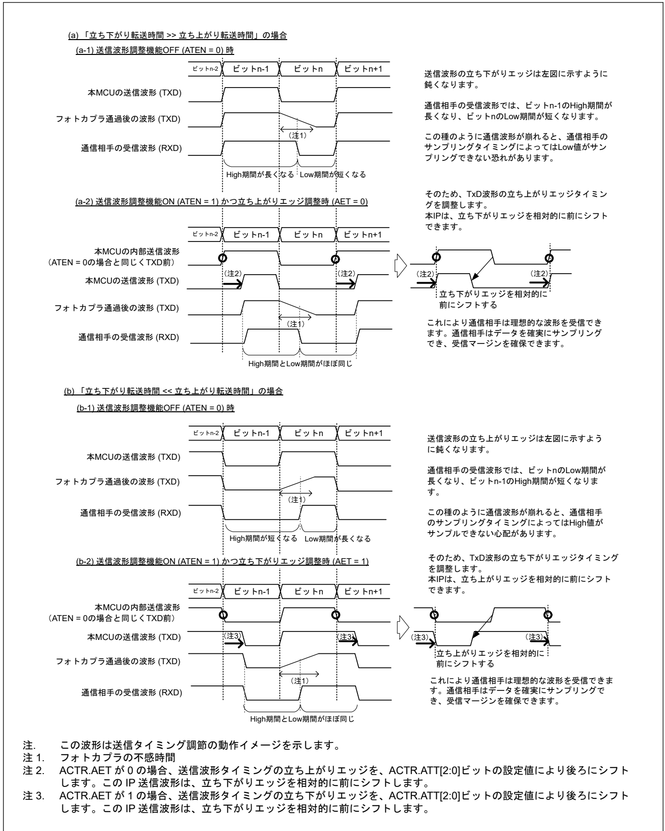
図 29.36 フォトコピラを通過する通信の送信動作の概要
