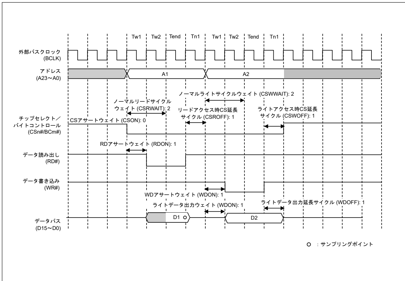
図 14.9 ノーマルアクセスの動作例（読み出し、書き込み）（ n = 0 \sim 7 、 m = 0 \sim 1 ）
