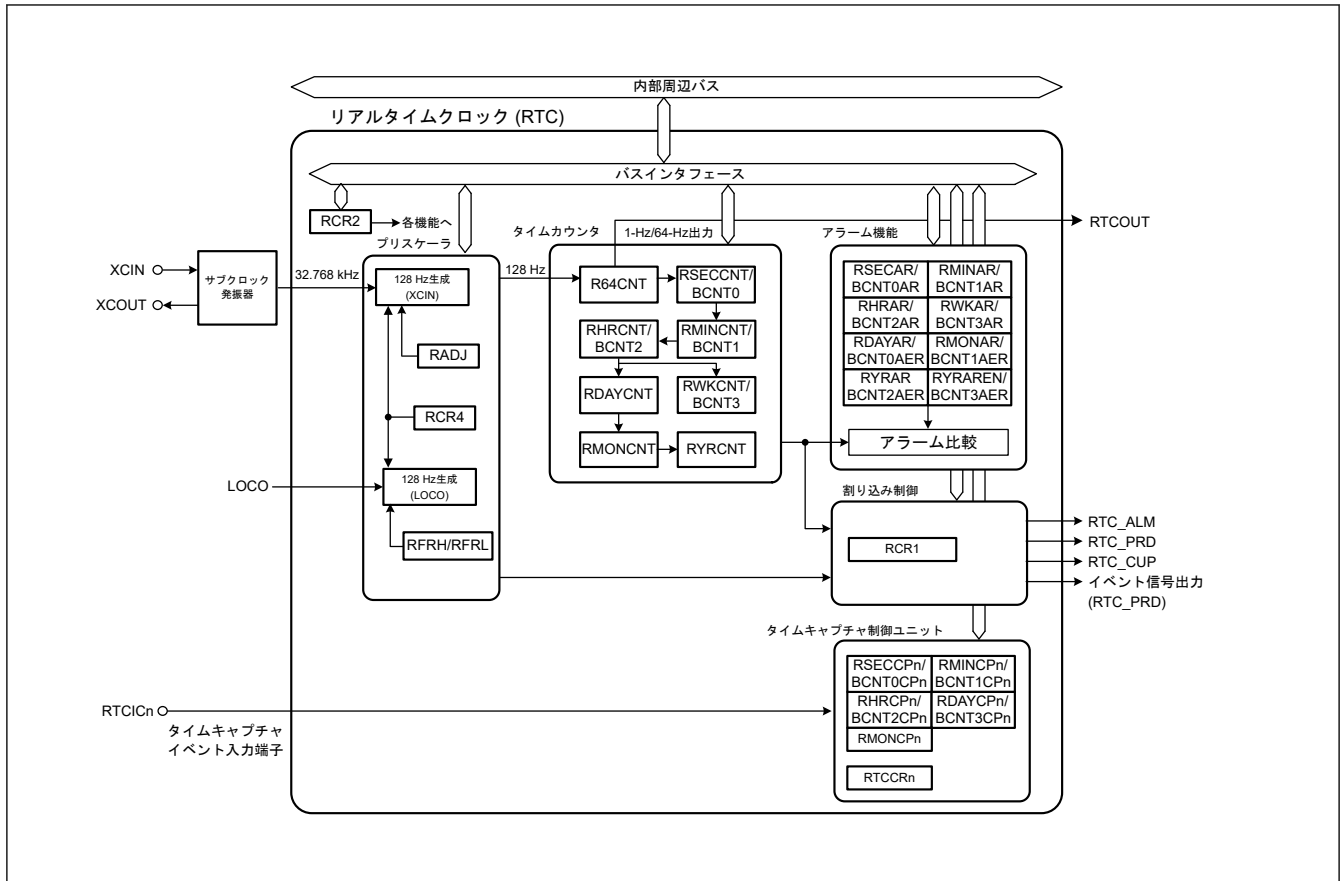
図 23.1 RTC のブロック図
