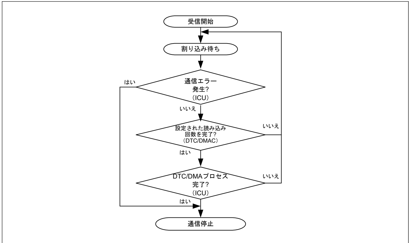
図 35.55 受信手順
