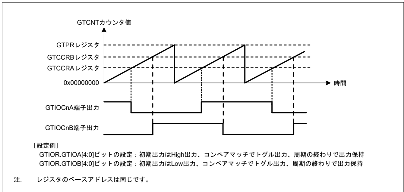
図 21.8 トグル出力動作例 (1)
