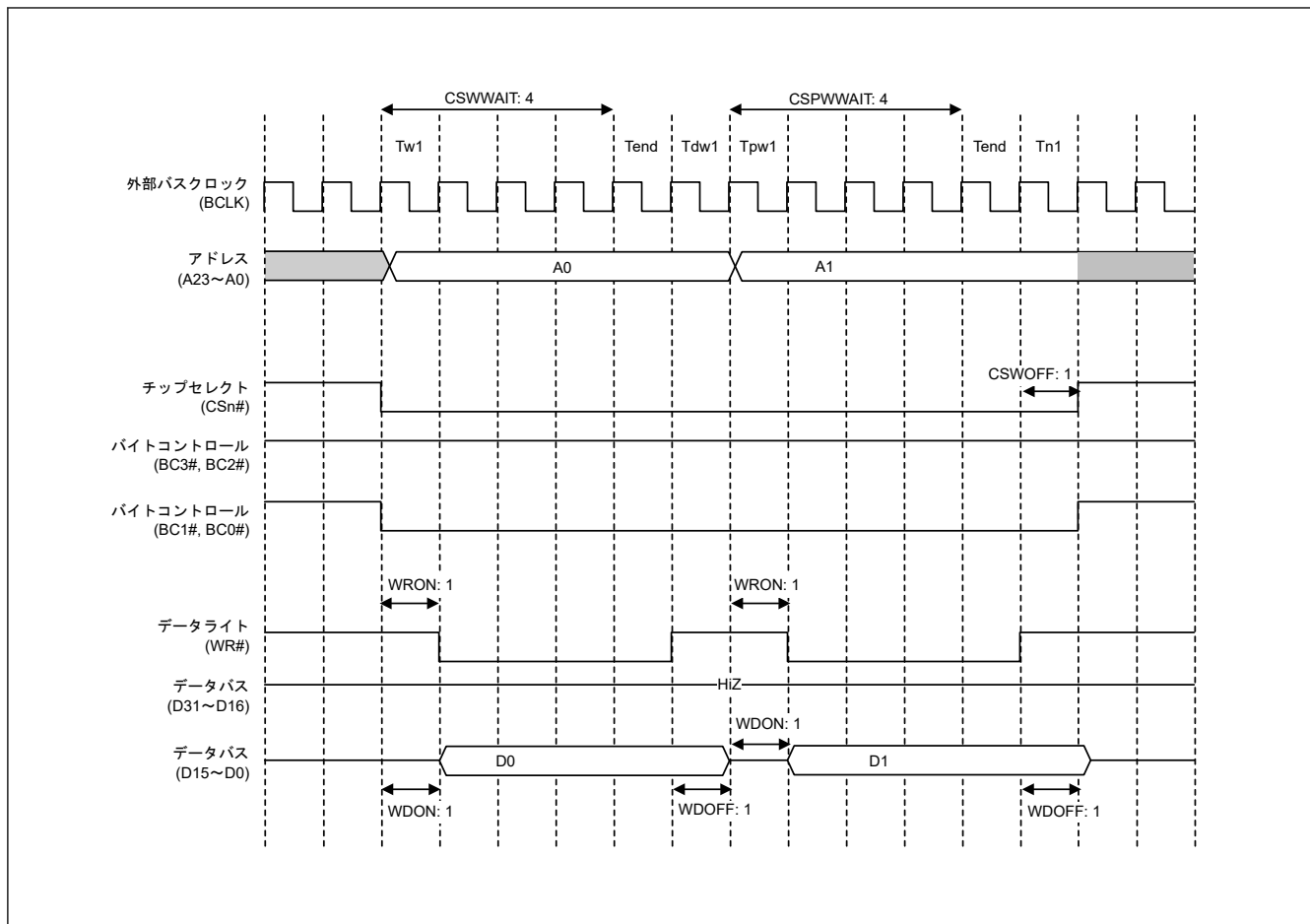
図 14.20 ページライトアクセスの動作例 (16 ビットバス空間に対する 32 ビットアクセスの場合、1 ライトストロープモード時) (n = 0~7)
