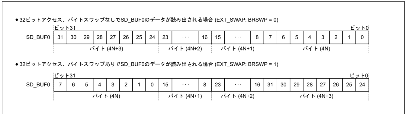
図 36.6 SD_BUF0 からの読み出し
