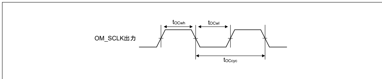
図 50.51 クロックタイミング
