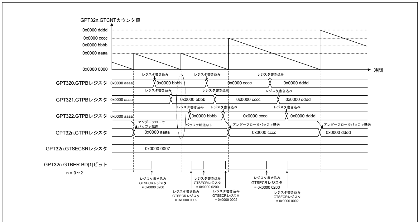
図 21.65 バッファ動作禁止の複数チャンネルの動作例（のこぎり波、シングルバッファ動作）
