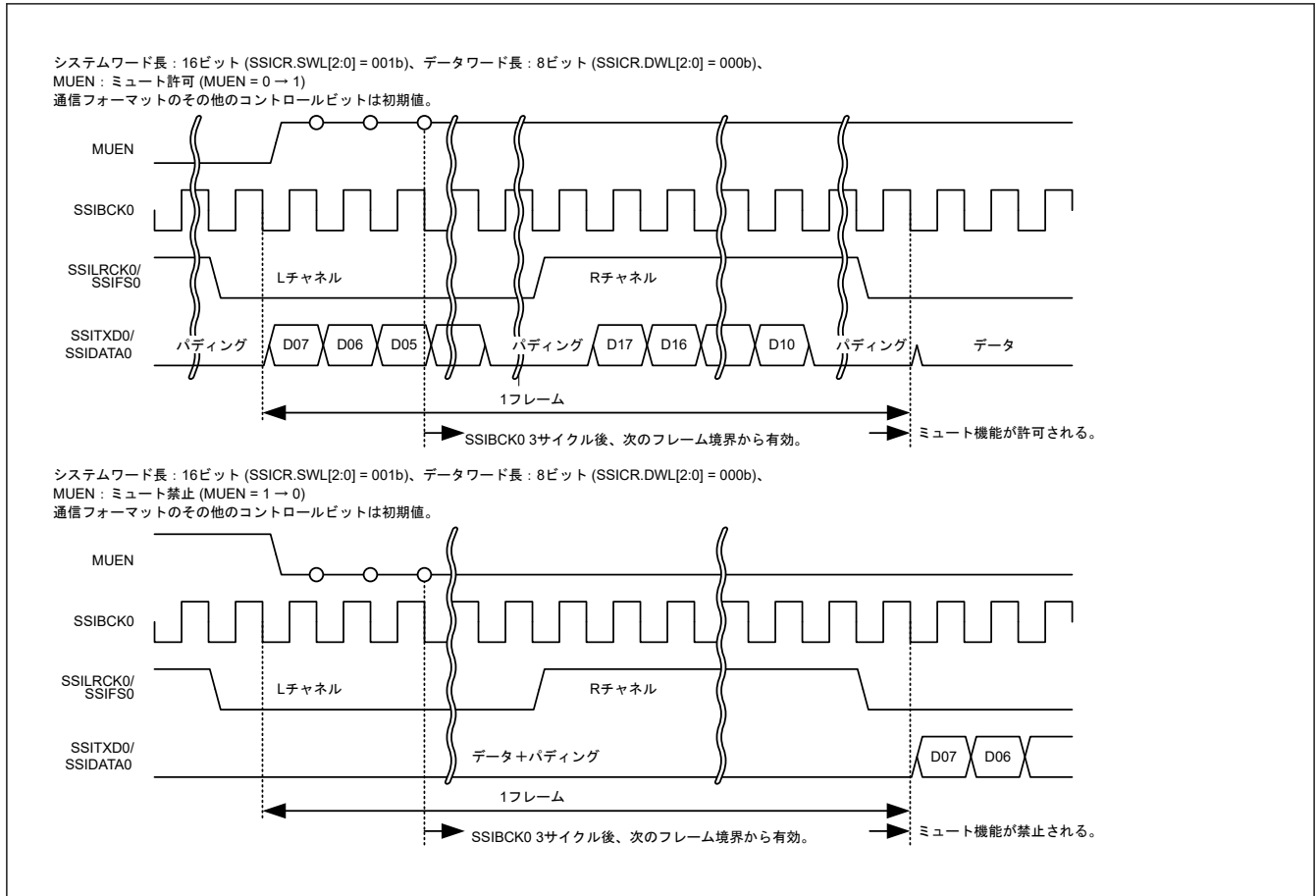
図 35.5 ミュート機能設定時のデータ送信
