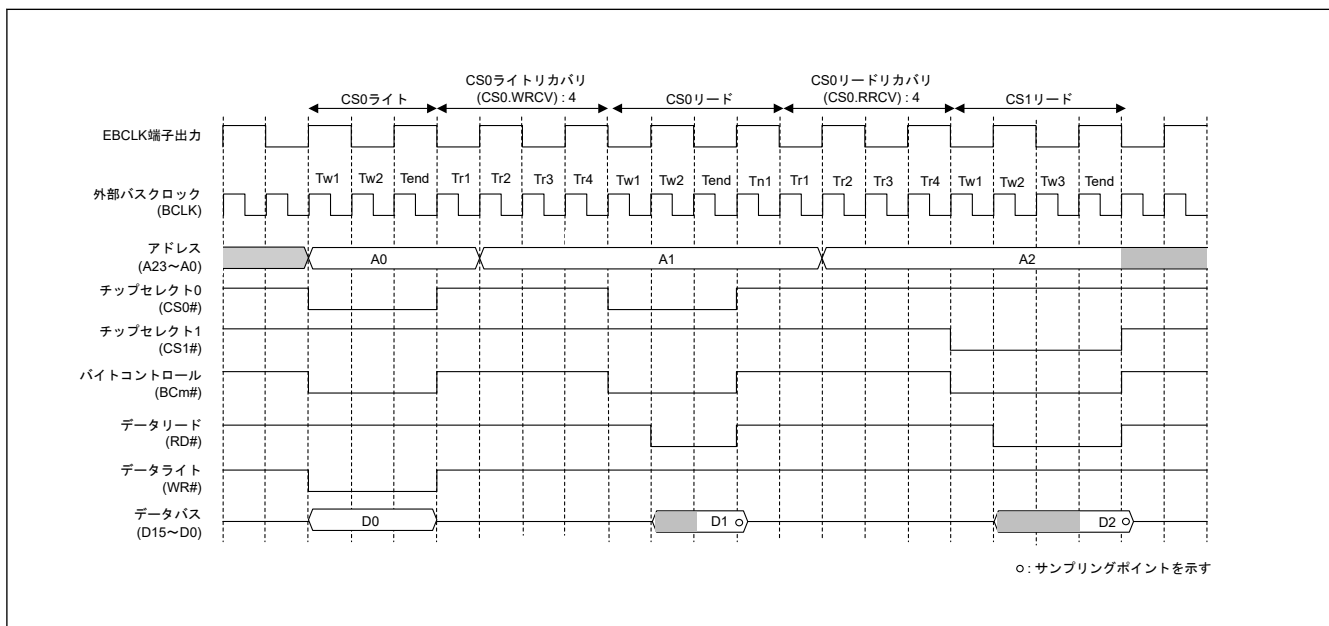
図 14.34 EBCLK 端子出力選択ビットで BCLK の 2 分周を選択した場合のリカバリサイクルの動作例（セパレートバスインターフェースによるノーマルアクセスの場合）(m = 0~1)
