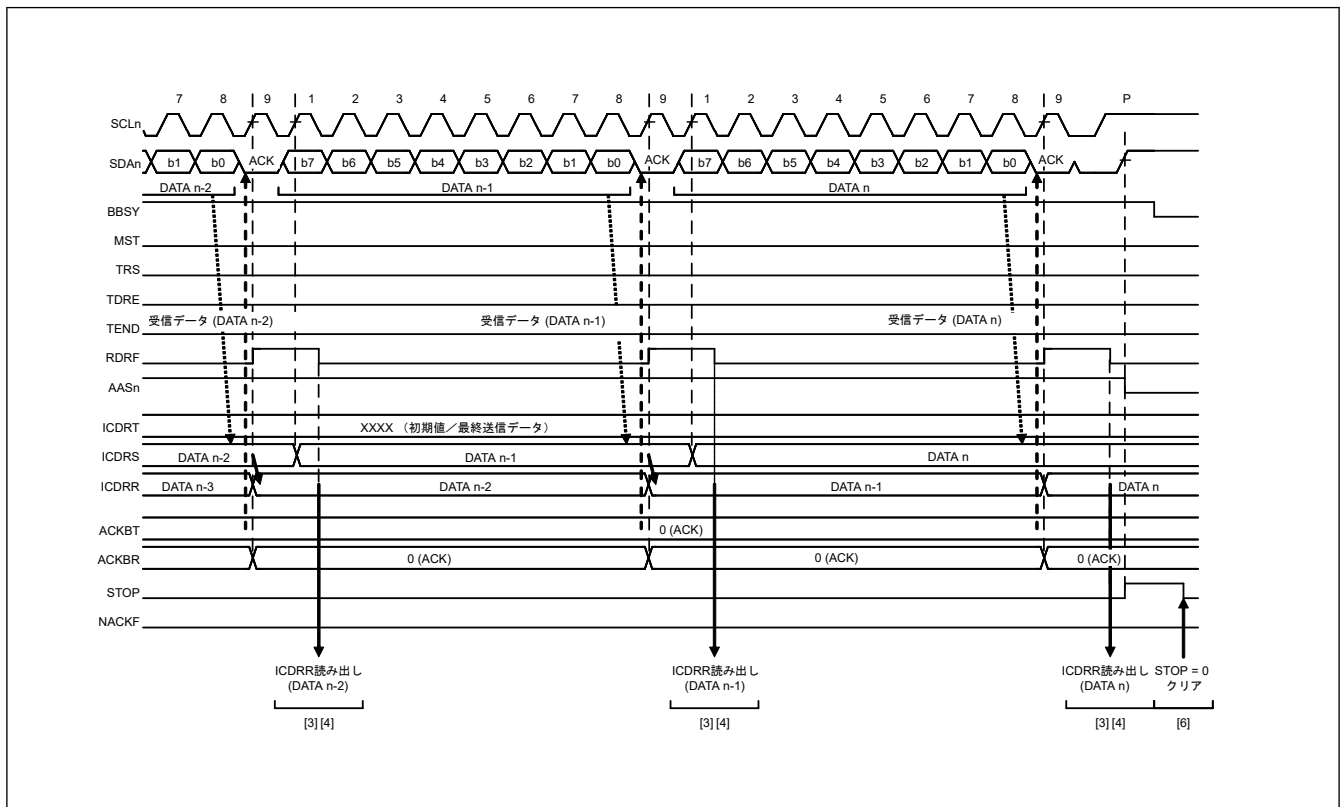
図 30.20 スレープ受信の動作タイミング (2) (RDRFS = 0 の場合)
