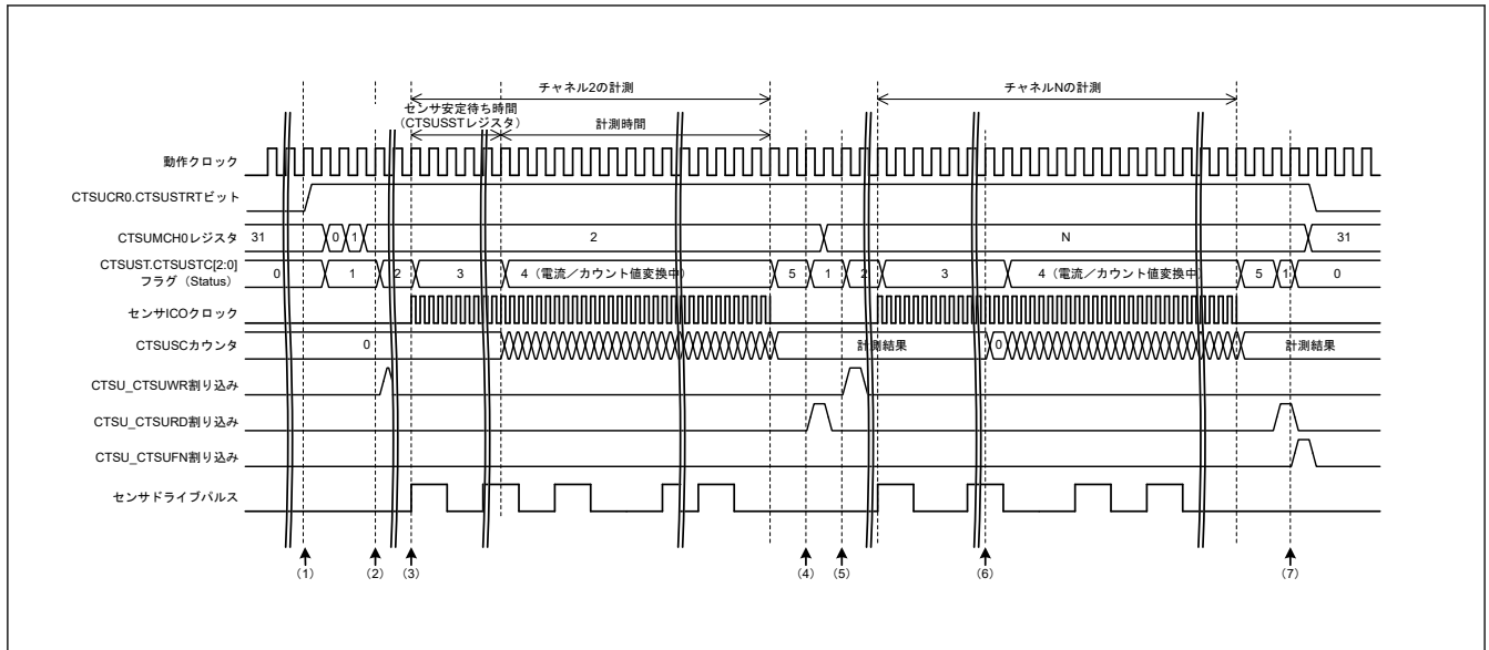
図 43.15 自己容量マルチスキャンモードのタイミング (計測開始条件がソフトウェアトリガの場合)
