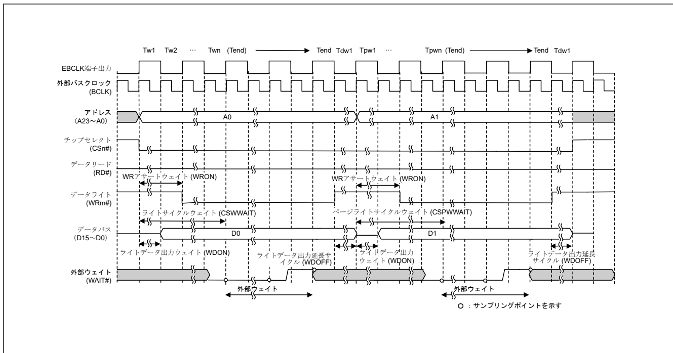
図 14.29 バイトストローブモード時の 16 ビットバス空間に対するページライトアクセスの外部ウェイトタイミング例 (EBCLK 端子出力選択ビットで BCLK の 2 分周を選択した場合) (n = 0~7, m = 0, 1)
