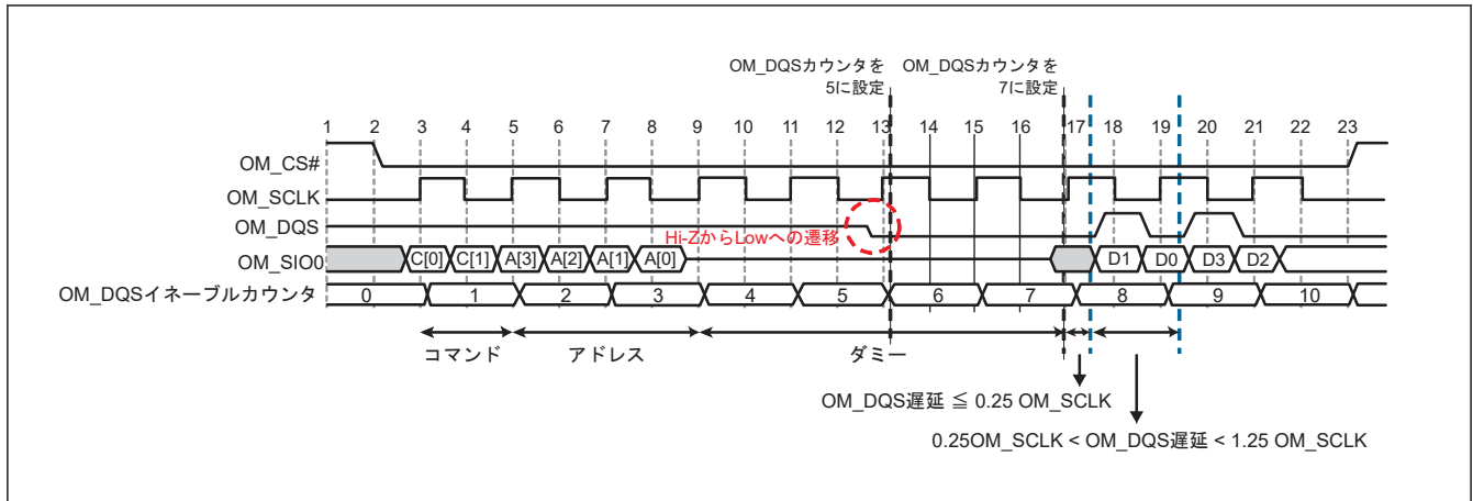
図 34.22 OM_DQS クロック入力が Hi-Z から Low に遷移するタイミングの例 (フラッシュ DOPI モード、ダミーサイクル数 = 4、OM_DQS プレサイクル ON)
