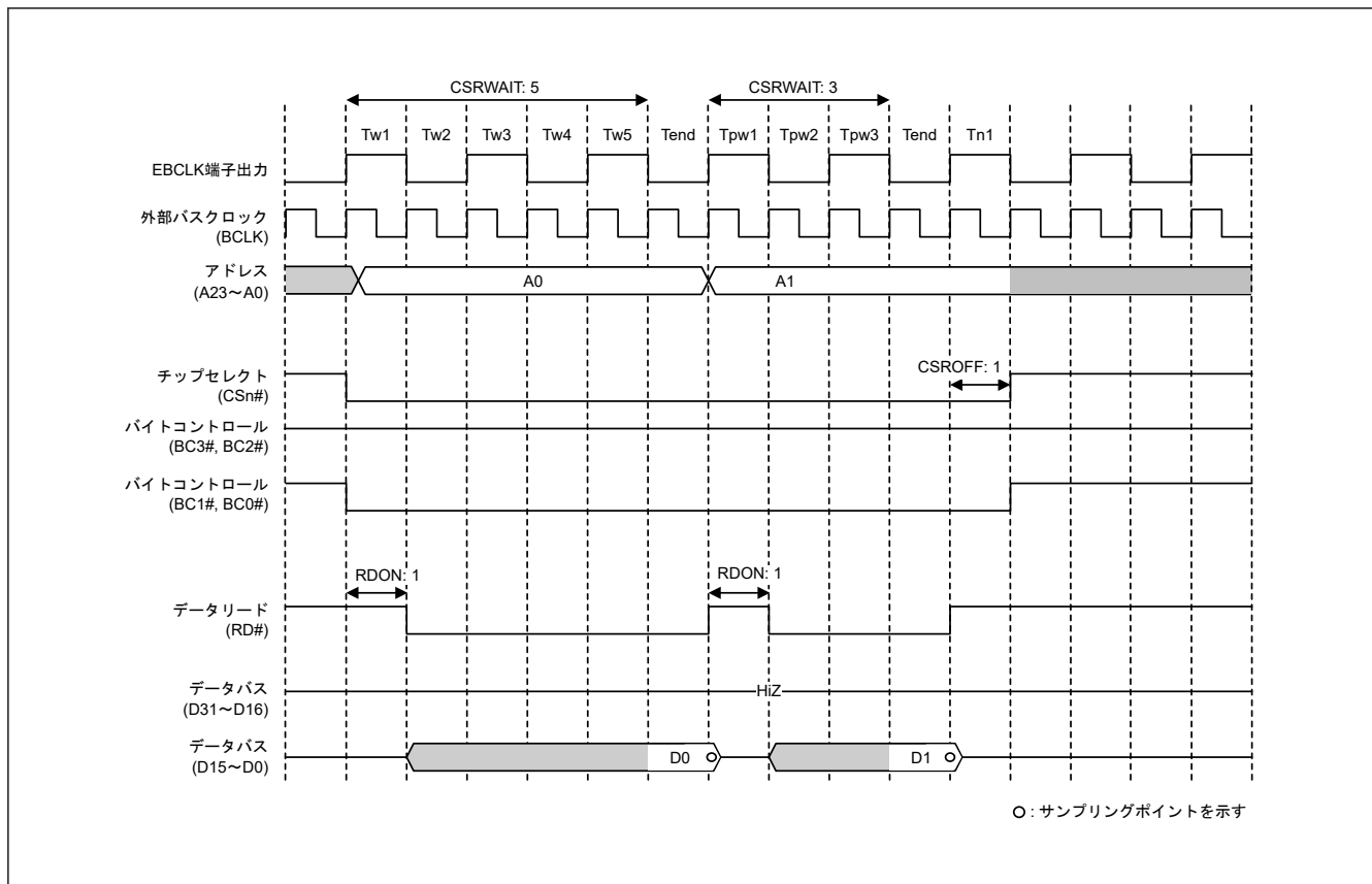
図 14.21 ページリードアクセスの動作例 (EBCLK 端子出力選択ビットで BCLK の 2 分周を設定した場合、および 1 転送要求に対して 2 回バスアクセスが発生する場合) (n = 0~7)
