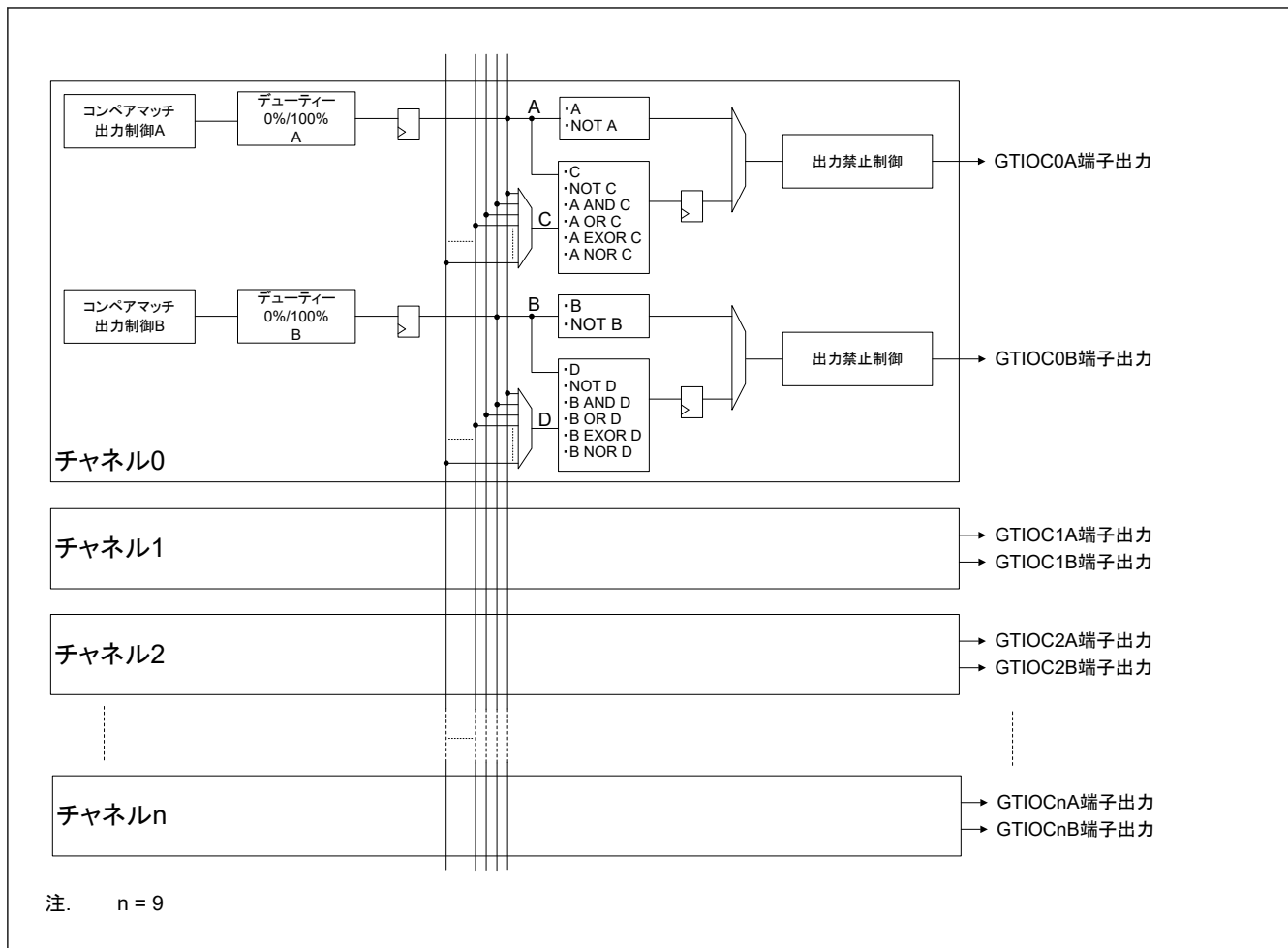
図 21.61 チャンネル間論理演算のブロック図 図 21.62 に、チャンネル間論理演算の例を示します。
