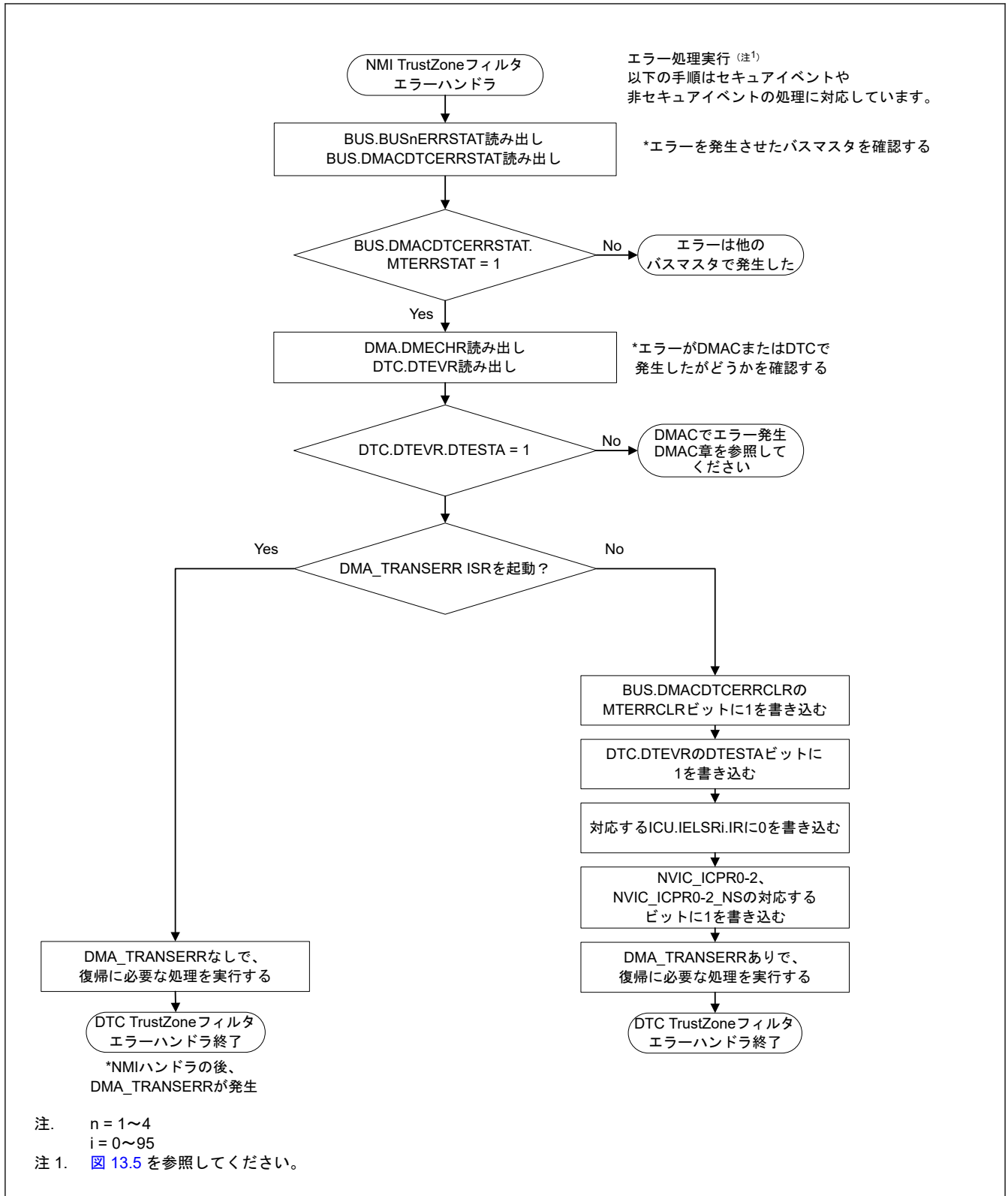
図 17.14 マスタ TrustZone フィルタエラーの NMI ハンドラにおける処理
