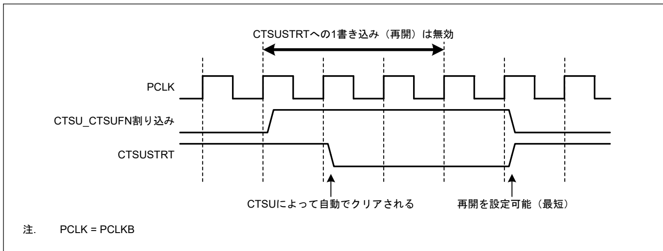
図 43.21 再開時の注意事項
