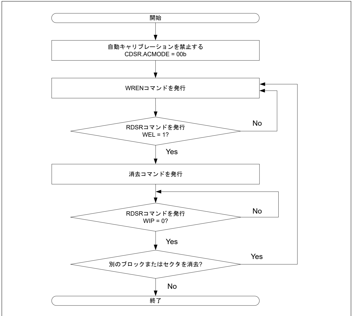
図 34.18 OctaFlash 消去の手順
