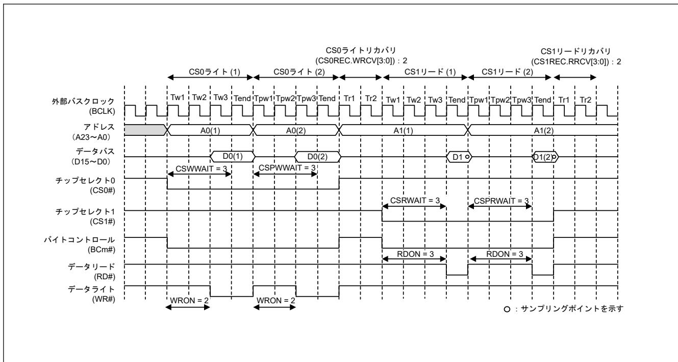
図 14.33 バスアクセスが分割された場合のリカバリサイクルの動作例（セパレートバスインターフェース、ページアクセスの場合）(m = 0~1)
