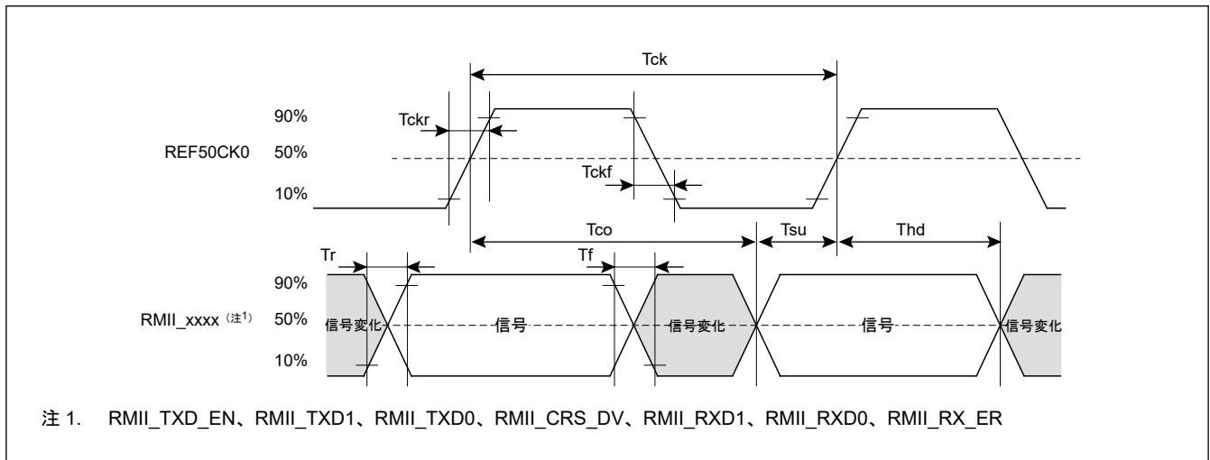
図 50.64 REF50CK0、RMII の信号タイミング
