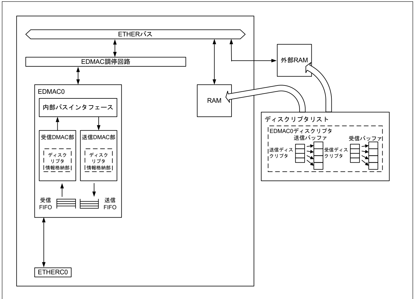
図 27.2 メモリ内のディスクリプタおよび送受信バッファの構成
