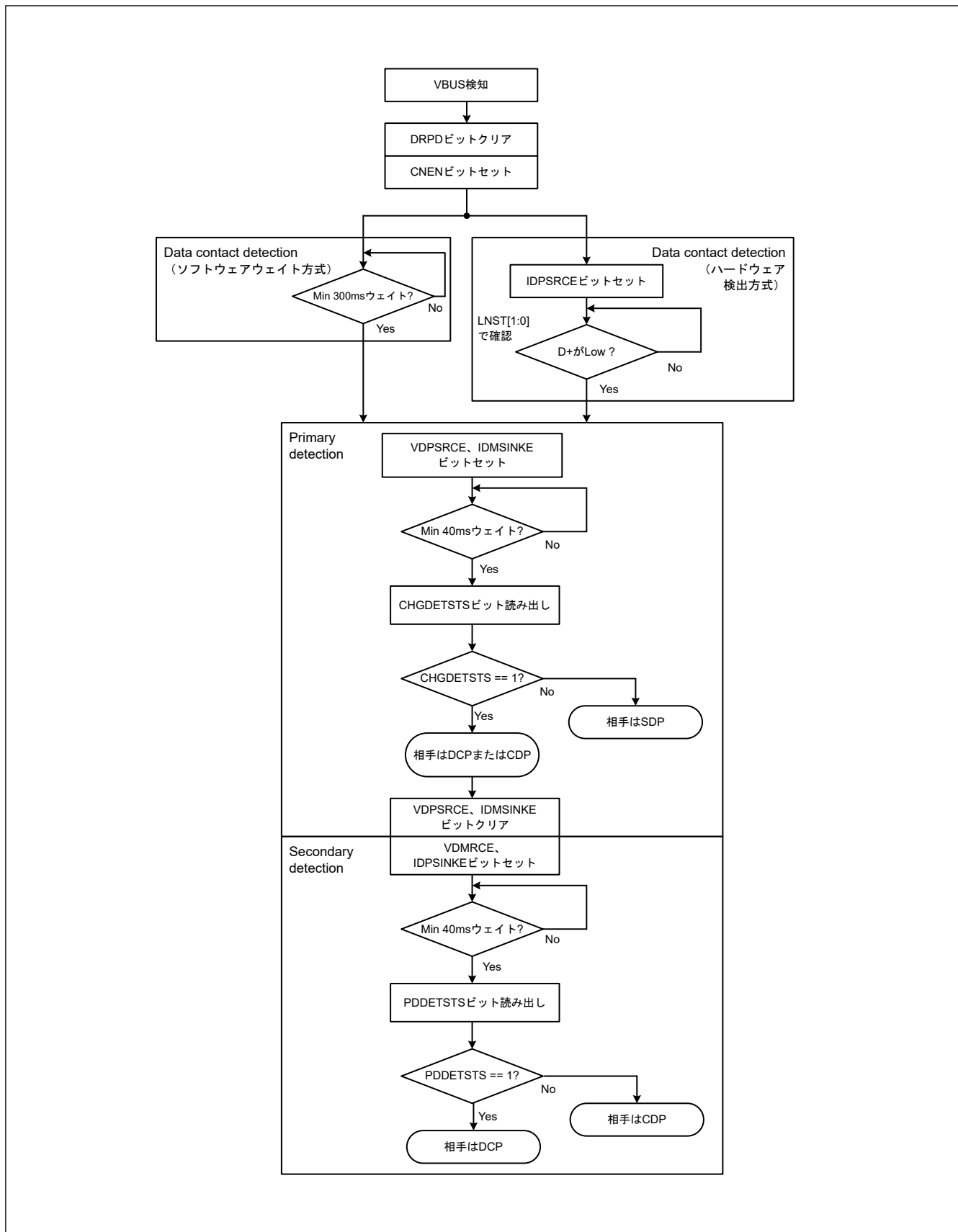
図 29.19 Portable Device としての処理フロー
