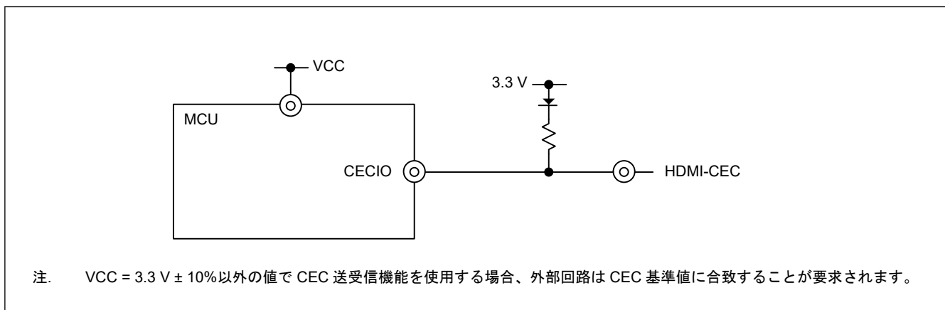
図 37.2 外部回路への I/O 端子の接続例 (VCC = 3.3 V ± 10%の場合)
