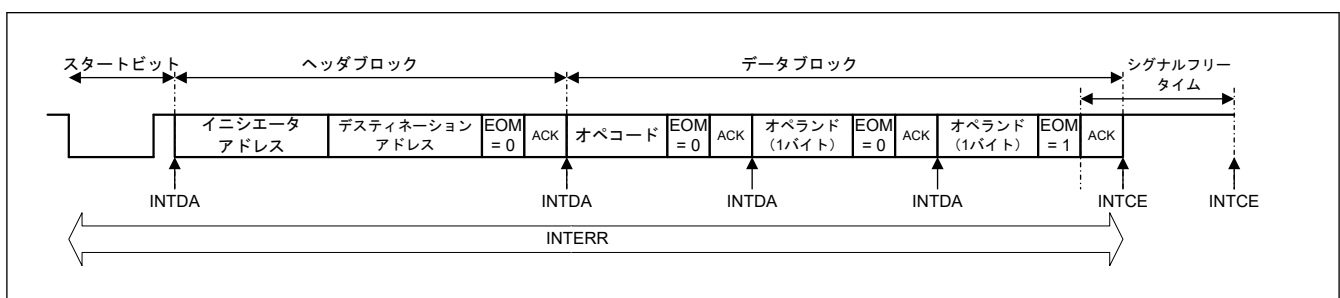
図 37.17 割り込みの発生タイミング
