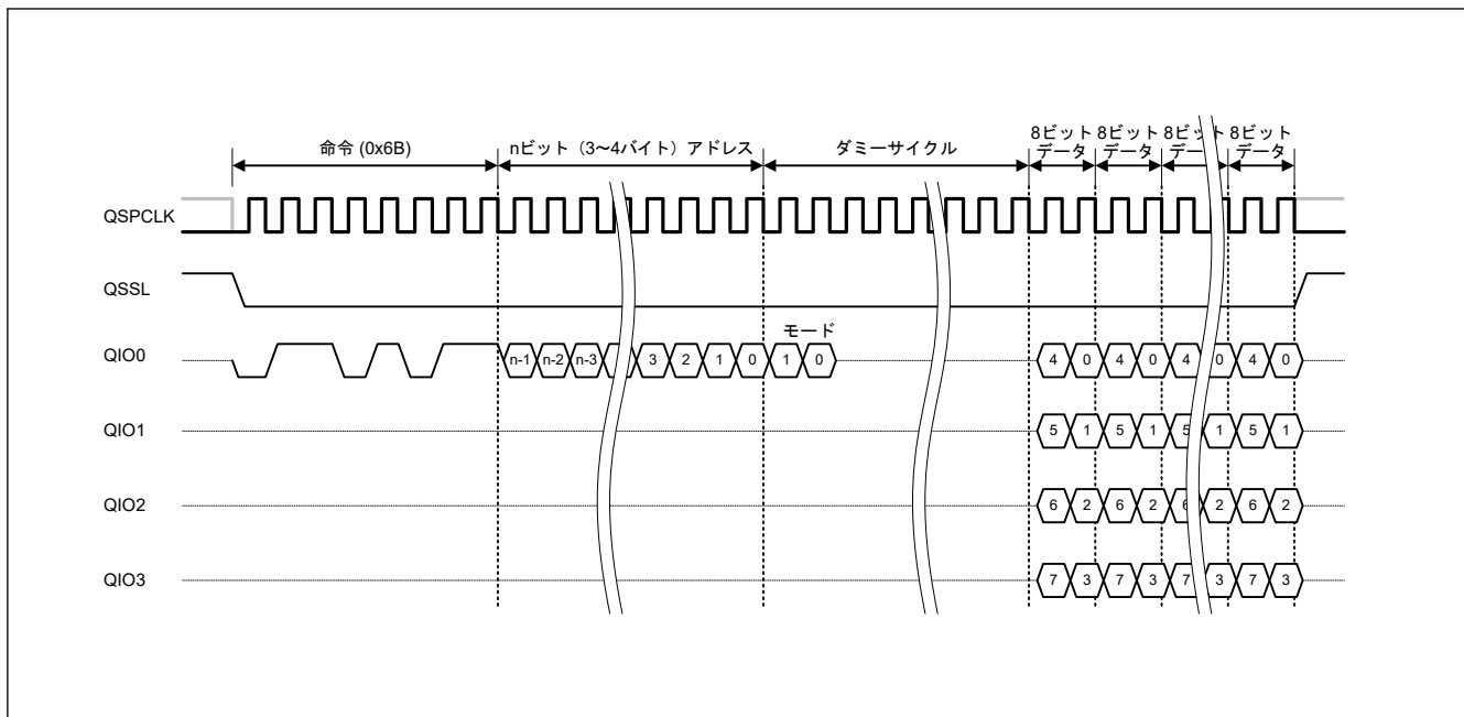
図 35.25 拡張 SPI プロトコルでのファストリード Quad 出力バスサイクル
