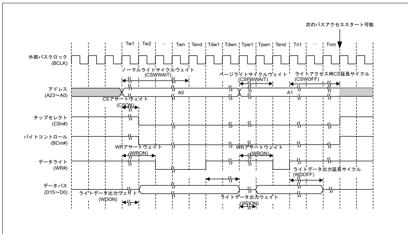
図 14.18 ページライトアクセスタイミング (n = 0~7、m = 0~1)
