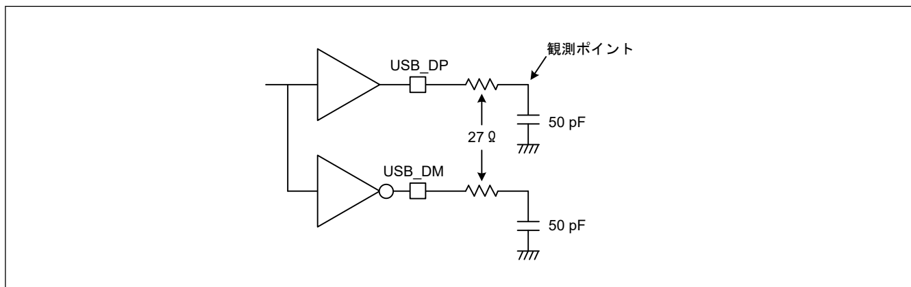
図 53.81 フルスピードモードにおける測定回路
