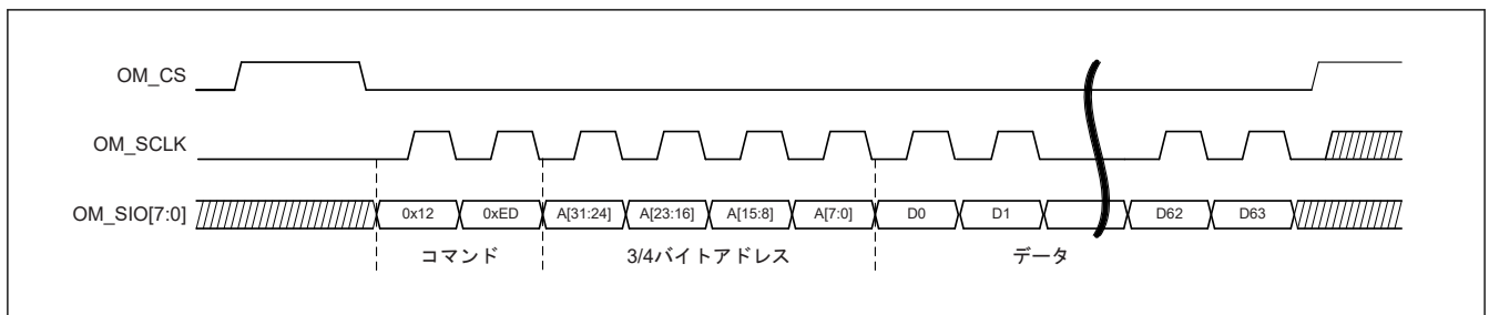
図 36.4 OctaFlash インタフェースでの書き込み動作の波形 (SOPI モード)
