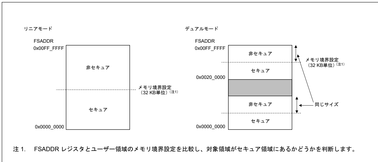
図 50.36 ユーザー領域のセキュア/非セキュア領域
