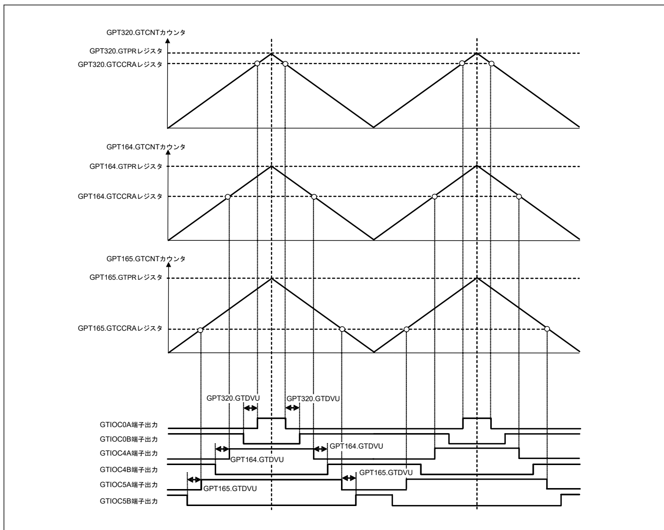
図 21.43 三角波 3 相相補 PWM 出力例 (デッドタイム自動設定)
