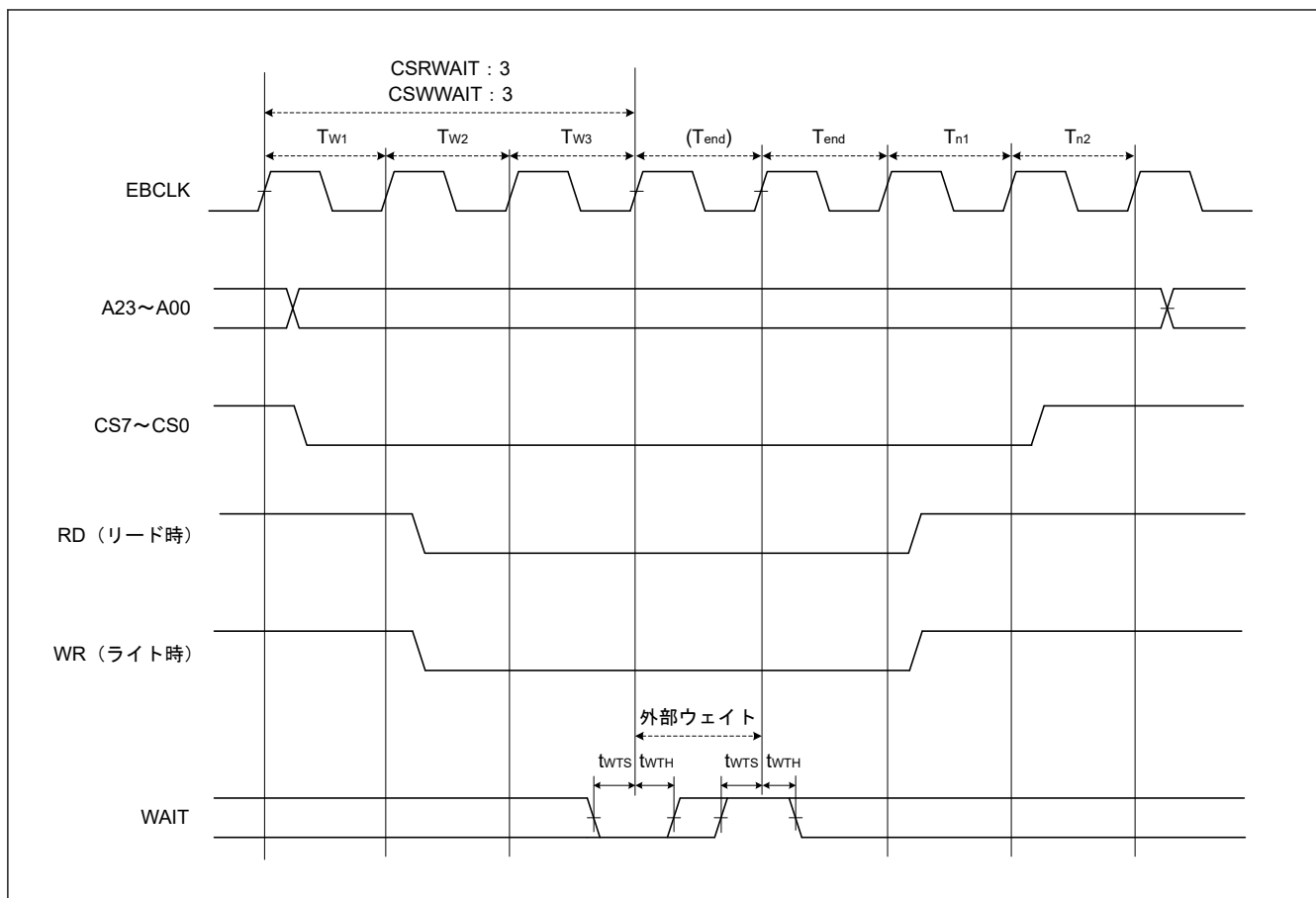
図 53.26 外部ウェイト制御の外部バスタイミング
