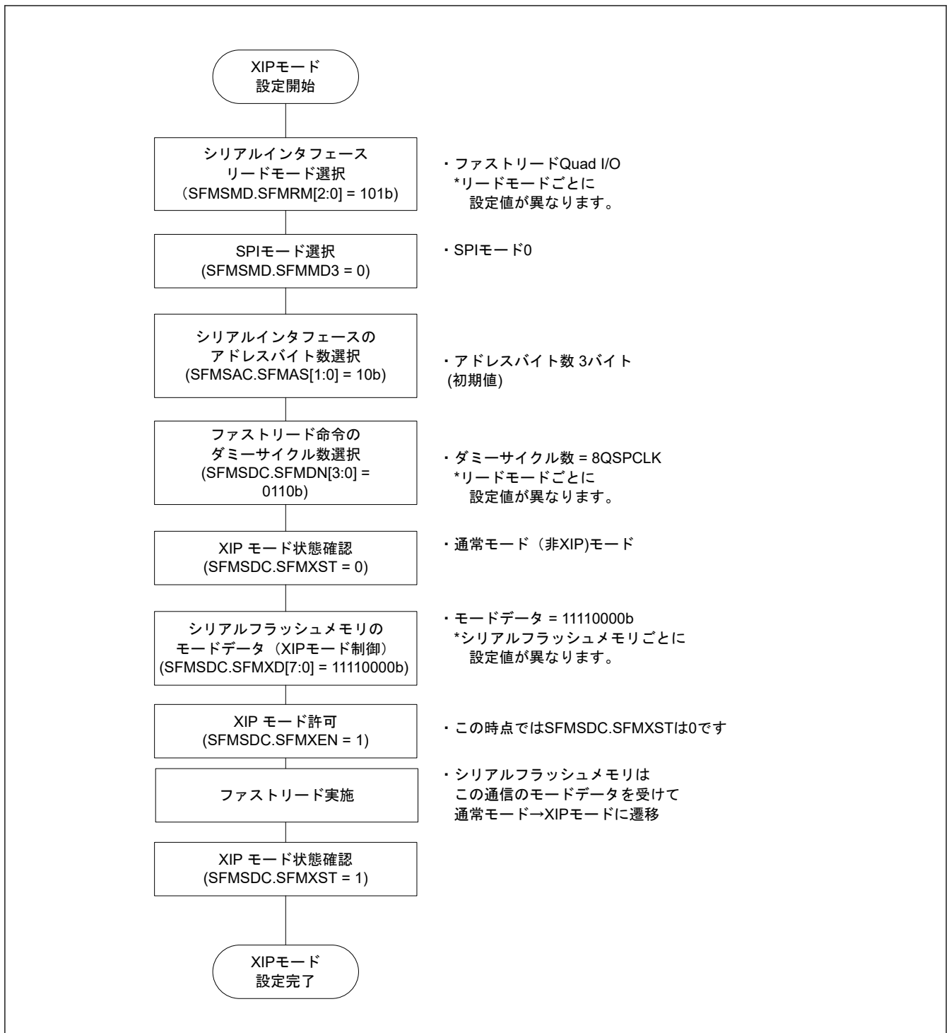
図 35.36 XIPモードのフローチャート
