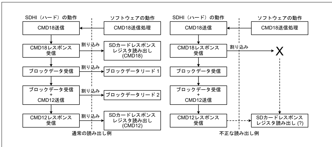
図 39.25 マルチブロックリード動作のフローチャート (2 ブロック)
