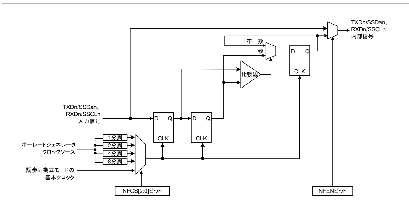
図 30.117 デジタルノイズフィルタ回路のブロック図
