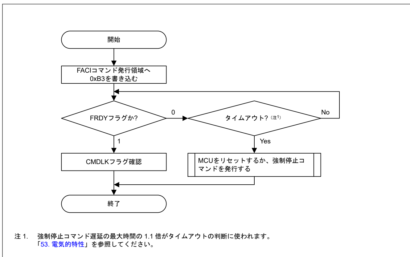
図 50.23 強制停止コマンドの使用フロー
