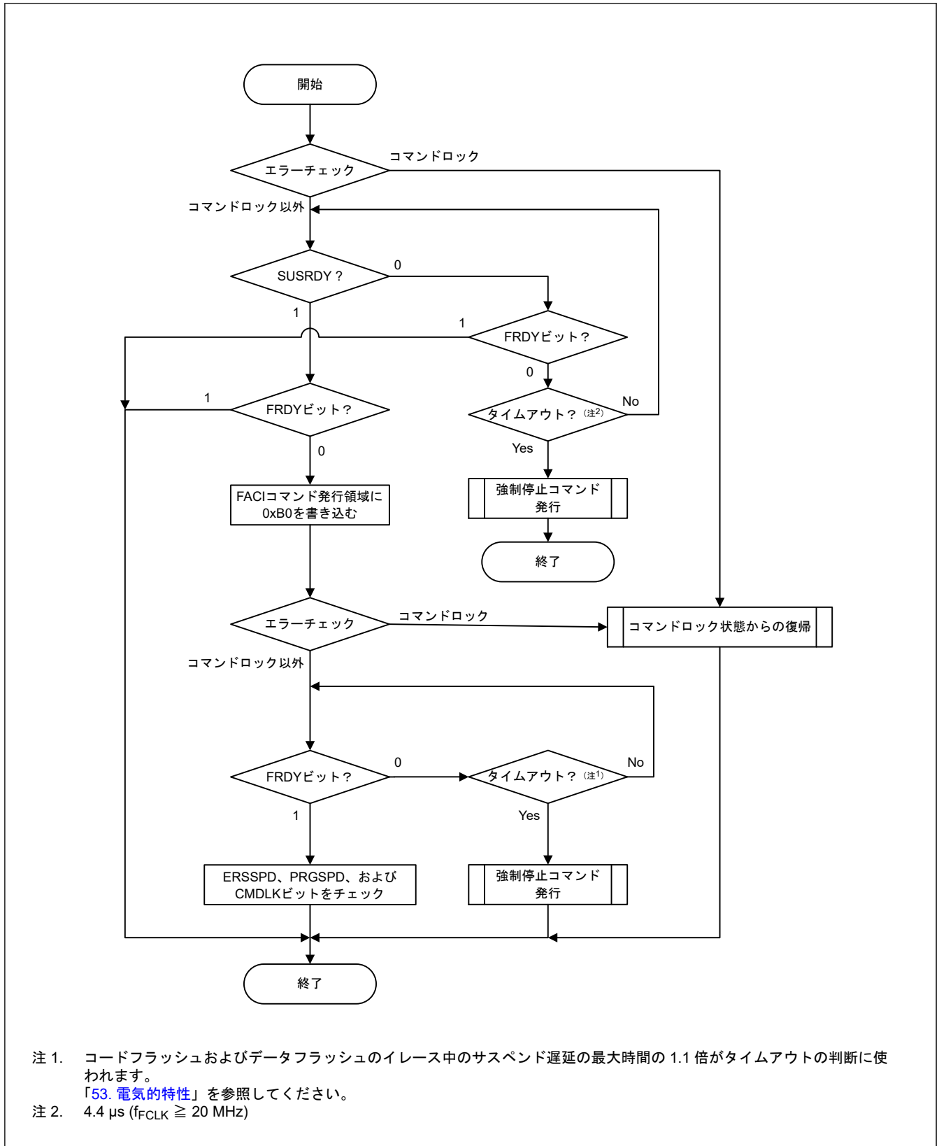
図 50.17 P/E サスペンドコマンドの使用フロー
