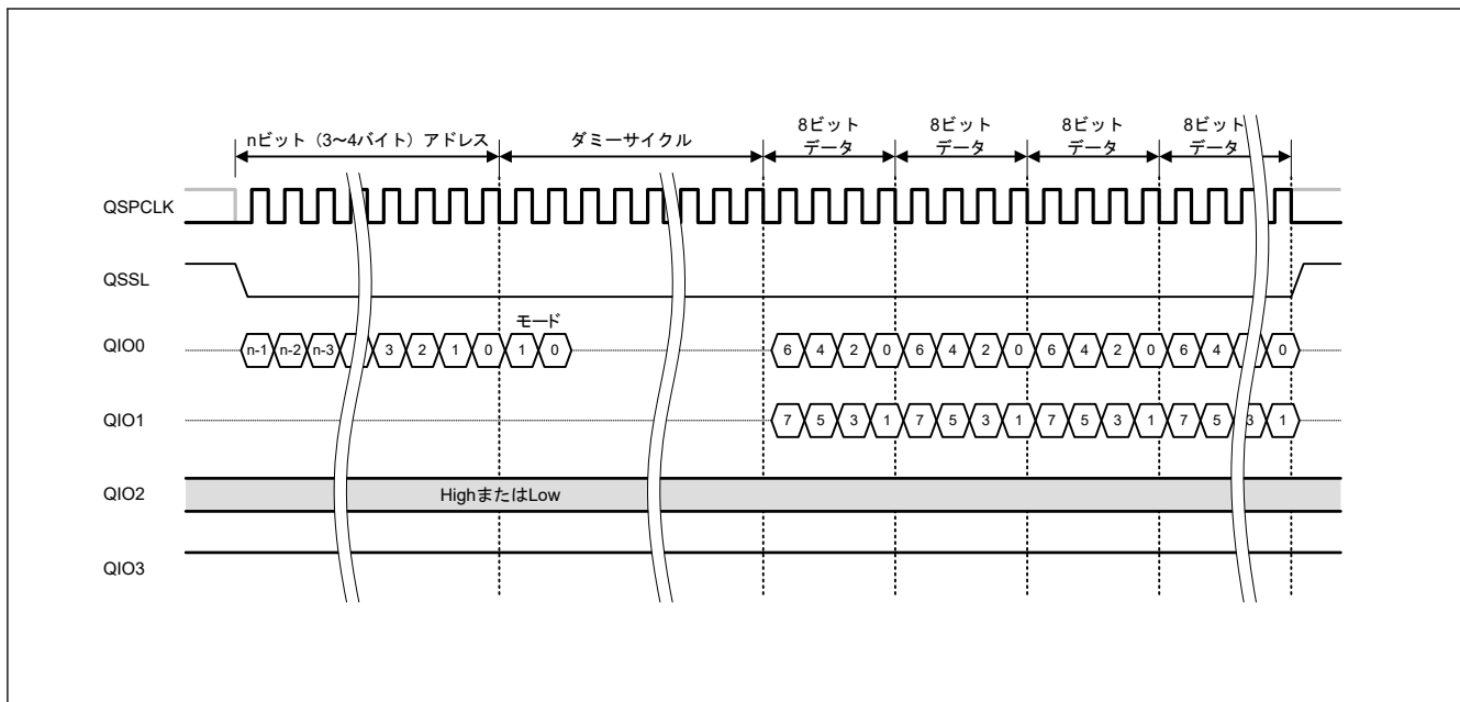
図 35.22 拡張 SPI プロトコルでの XIP モードファストリード Dual 出力バスサイクル
