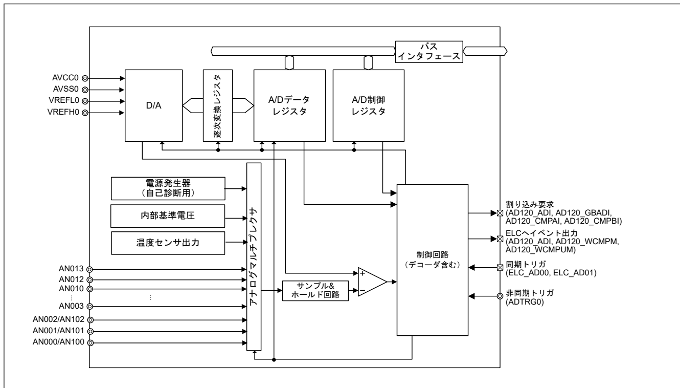
図 43.1 ADC12 のブロック図 (ユニット 0)
