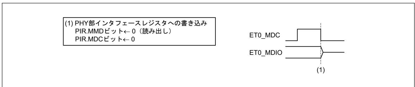
図 26.16 バス解放フロー (表 26.3 の読み出し動作時の TA)
