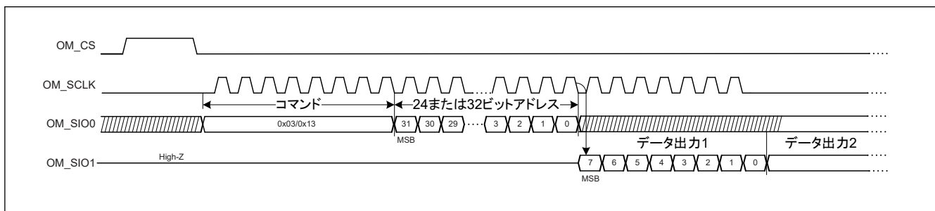
図 36.7 OctaFlash インタフェースでの読み出し動作の波形 (SPI モード)
