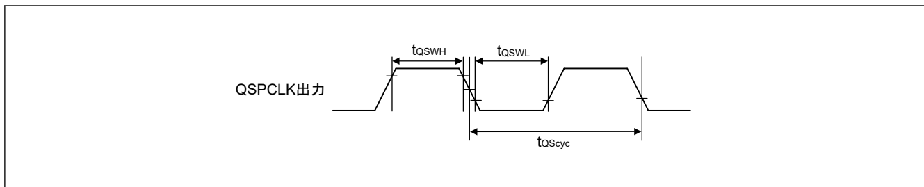
図 53.49 QSPI クロックタイミング
