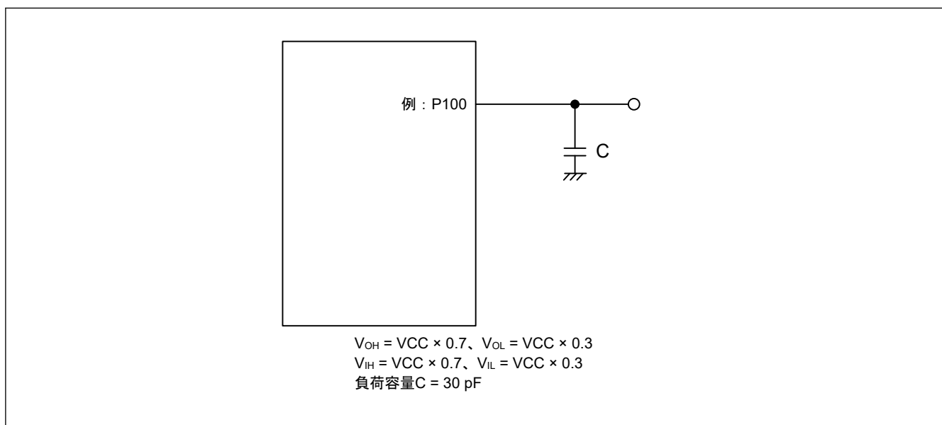
図 53.1 入出力タイミング計測条件
