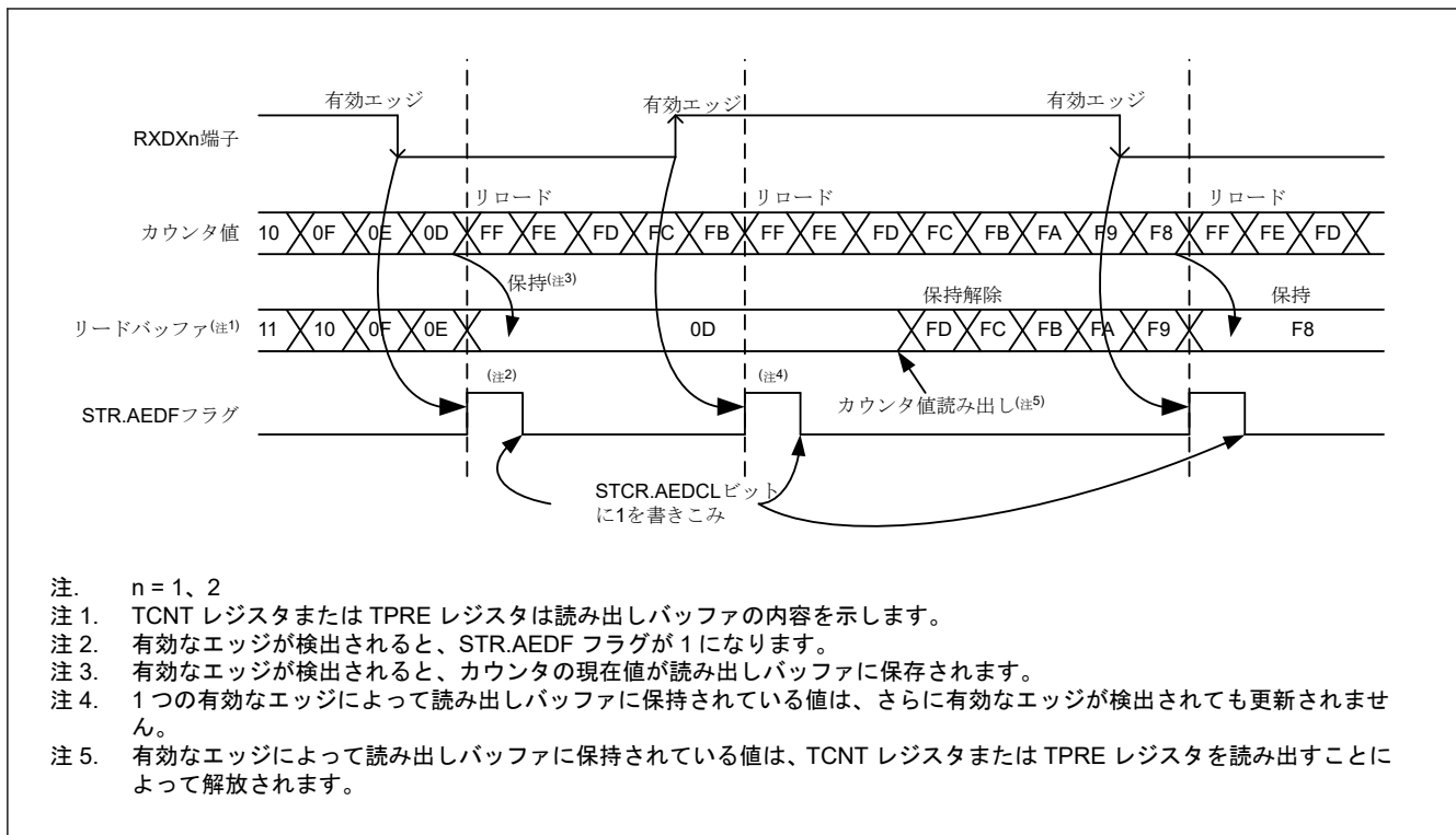
図 30.113 ビットレート測定機能動作例
