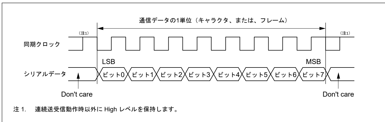
図 30.65 クロック同期式シリアル通信のデータフォーマット (LSB ファーストの並び順の場合)
