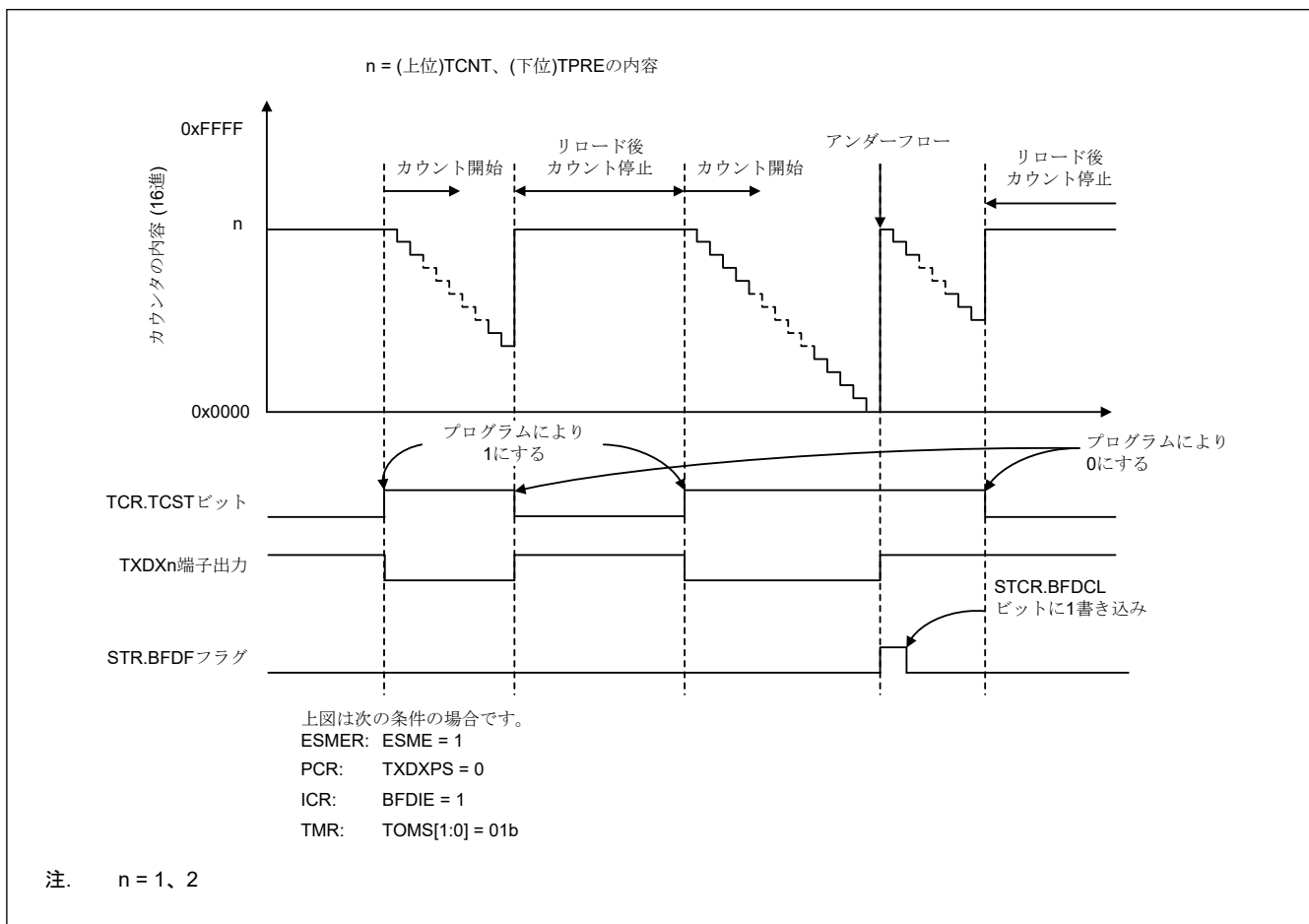
図 30.115 Break Field Low width 出力モードの動作例
