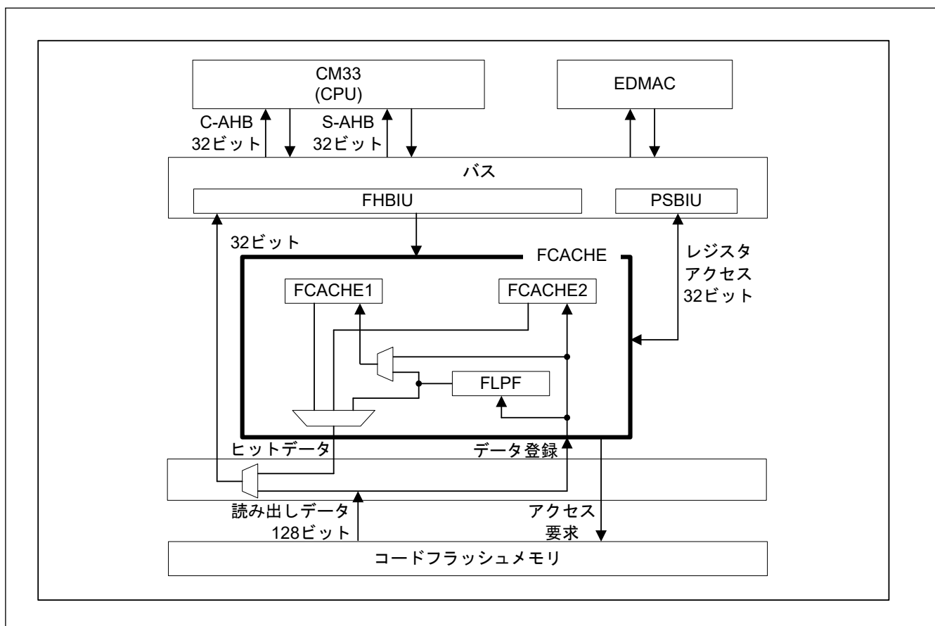
図 50.5 FCACHE のブロック図
