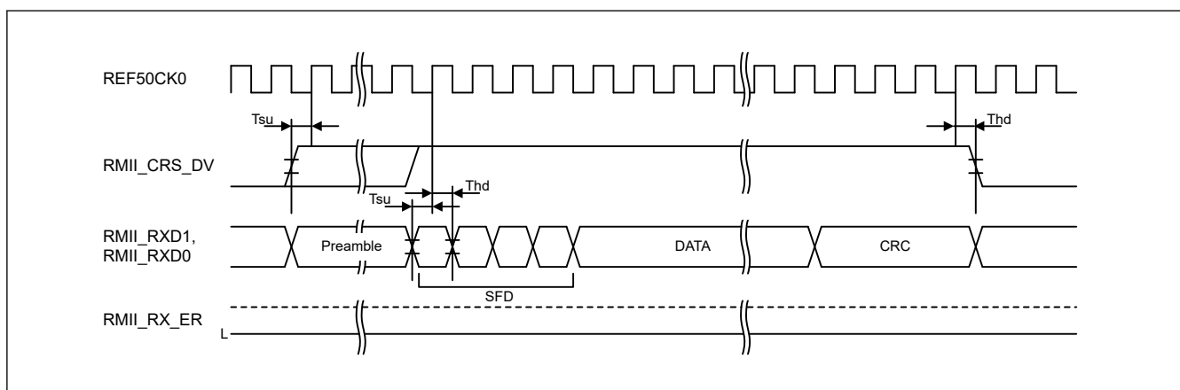
図 53.66 正常動作時の RMIi 受信タイミング
