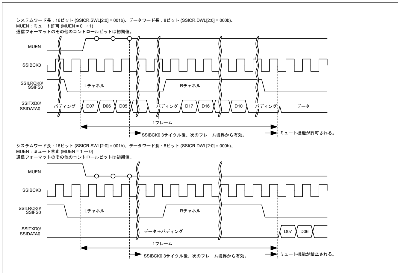
図 38.5 ミュート機能設定時のデータ送信
