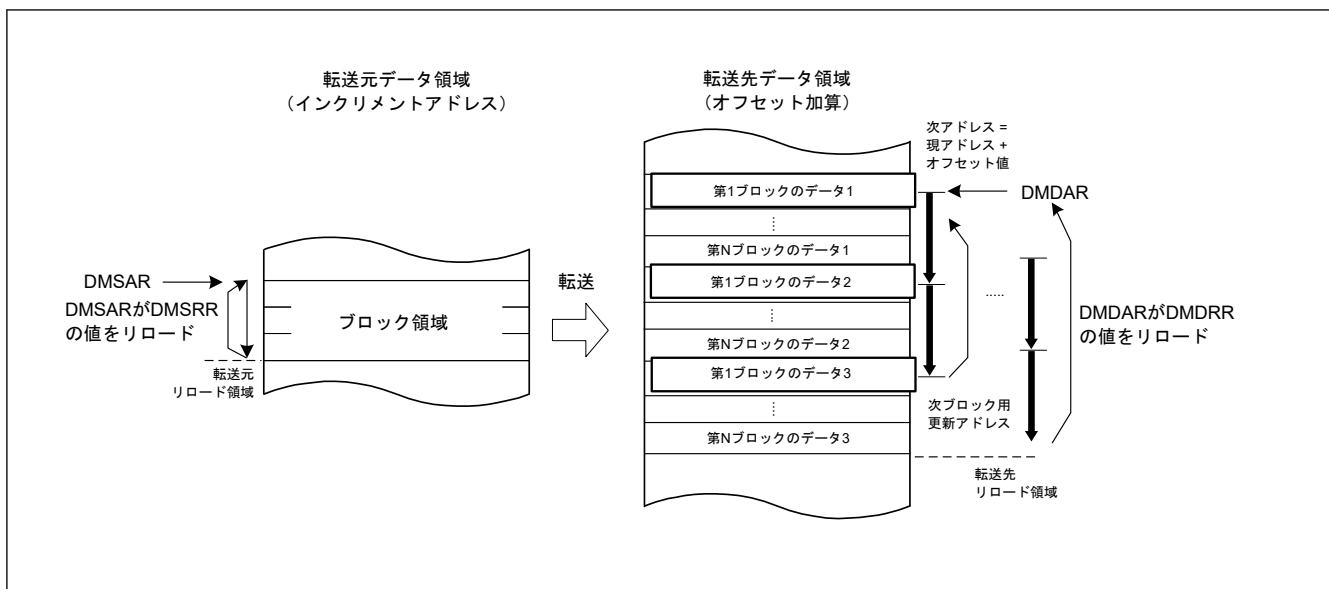
図 16.6 リピートブロック転送モードの動作 (オフセット加算)
