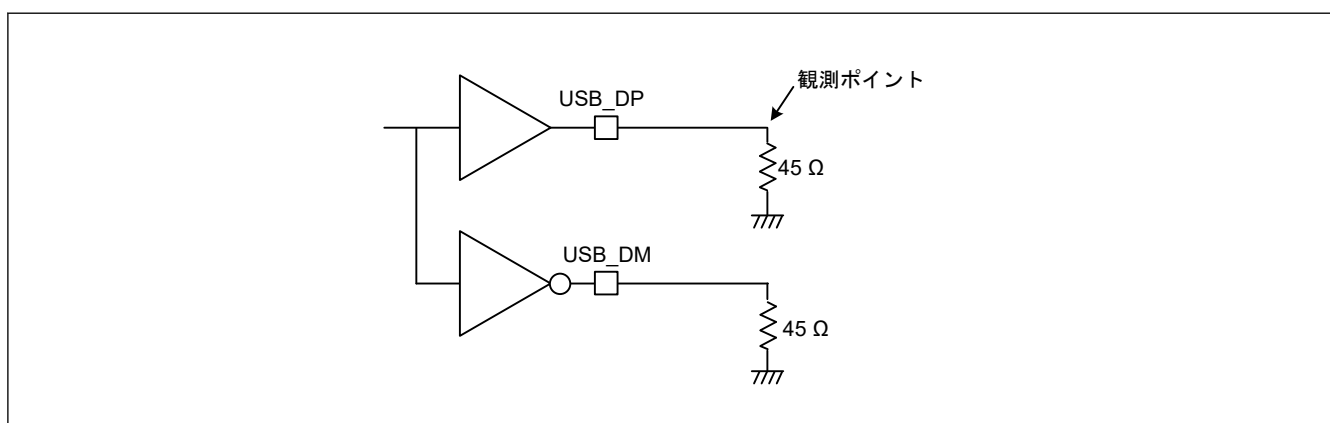
図 53.85 High-speed モードにおける測定回路
