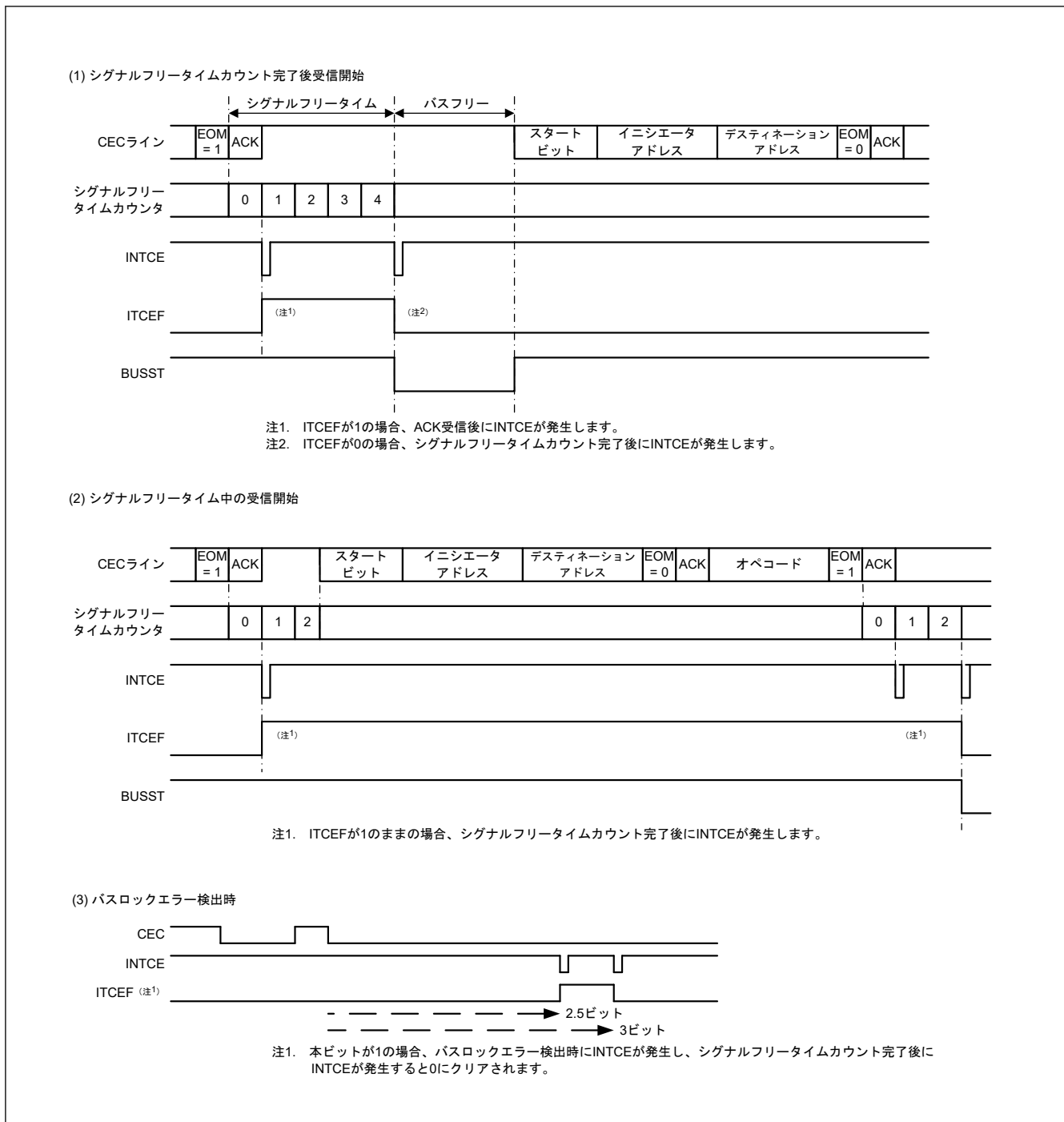
図 37.29 CECCTL1.CESEL[1:0] = 00b のときの ITCEF による INTCE 発生要因確認
