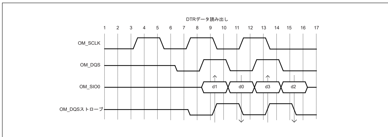
図 36.19 遅延 OM_DQS クロックを使用したデータのラッチ
