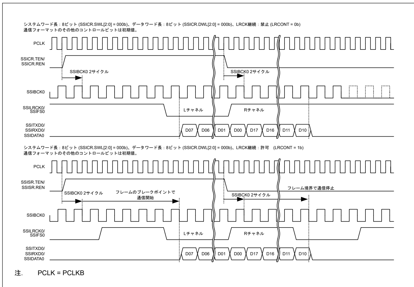
図 38.33 LR クロック/フレーム同期継続の動作例
