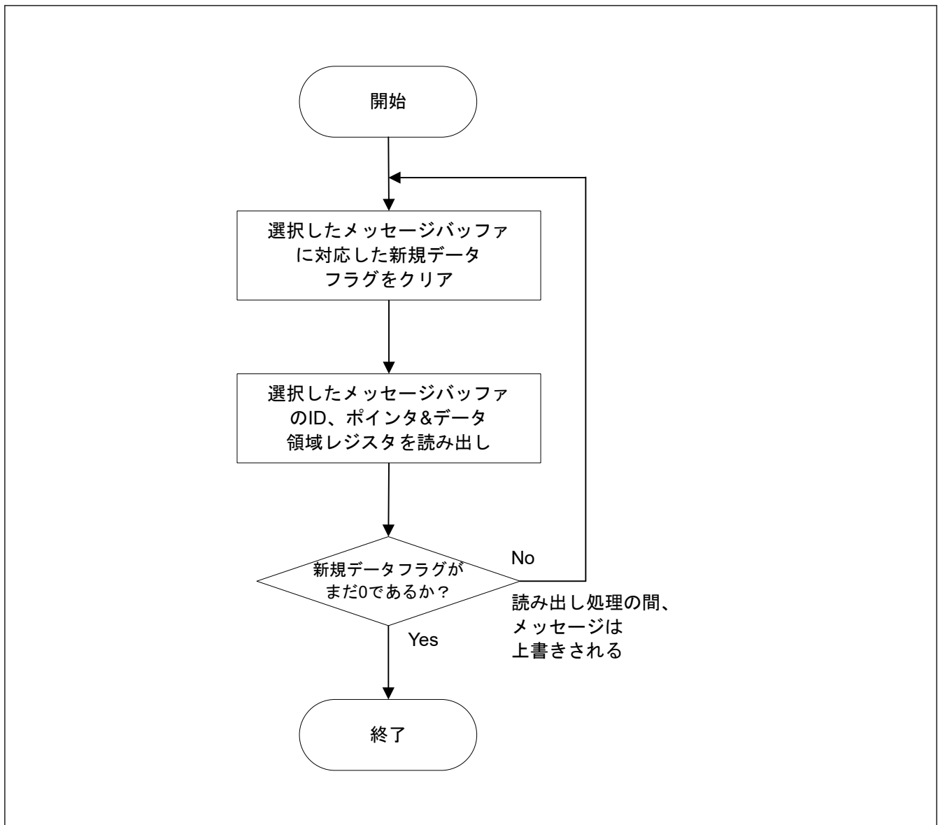
図 32.36 RX メッセージバッファの読み出し手順
