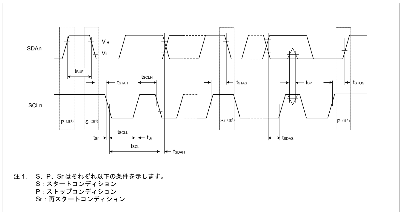
図 53.57 I 2 C バスインタフェース入出力タイミング
