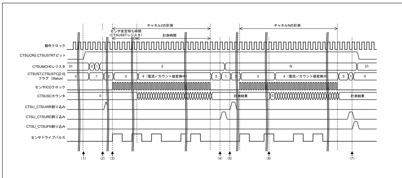
図 46.15 自己容量マルチスキャンモードのタイミング (計測開始条件がソフトウェアトリガの場合)
