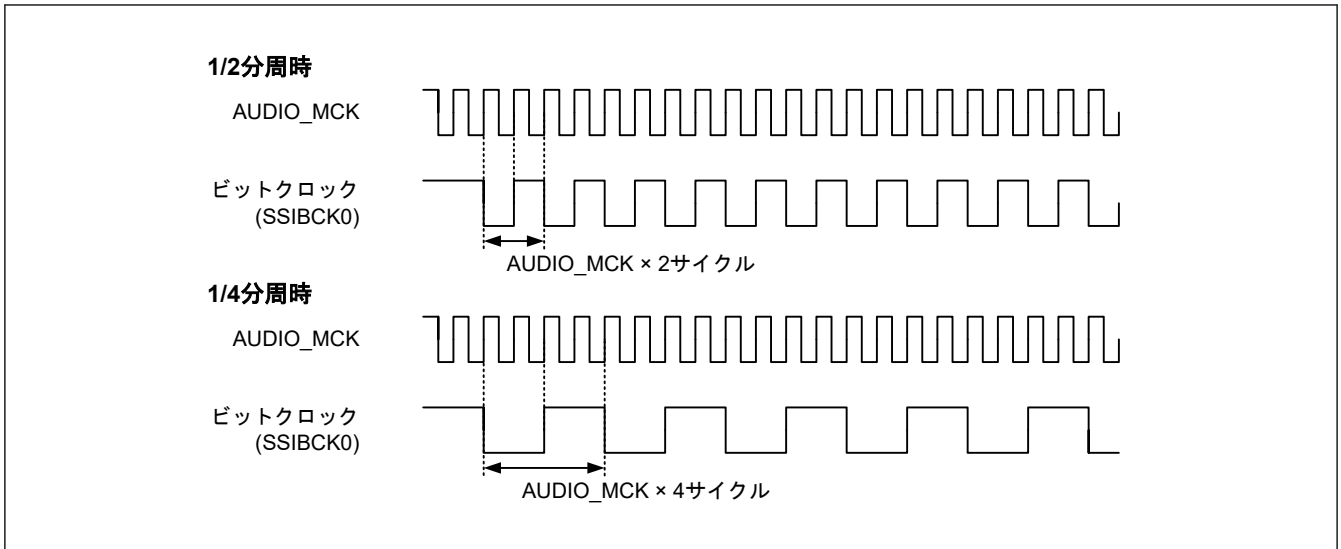
図 38.6 マスタモード通信時のサンプリング周波数
