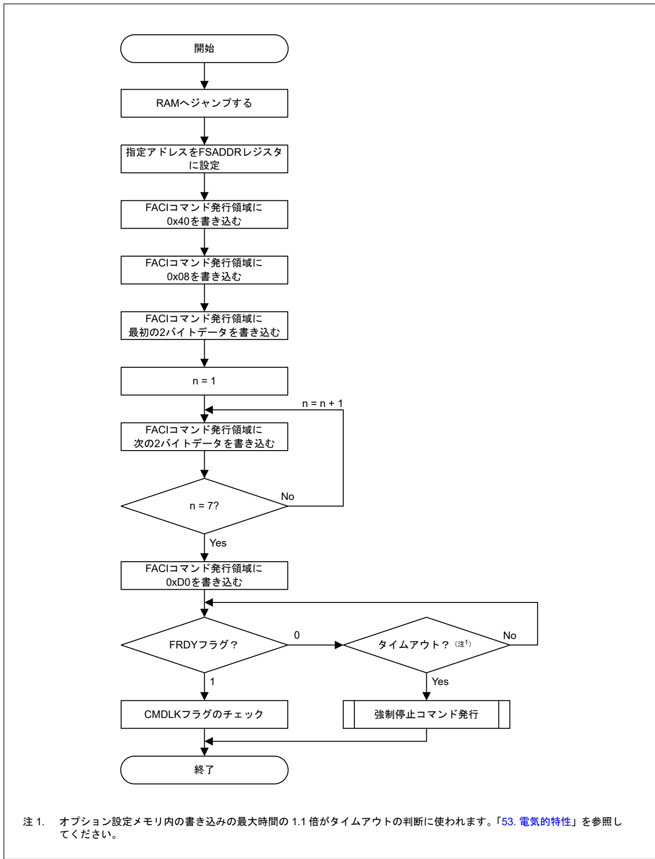
図 50.25 コンフィグレーション設定コマンドの使用フロー
