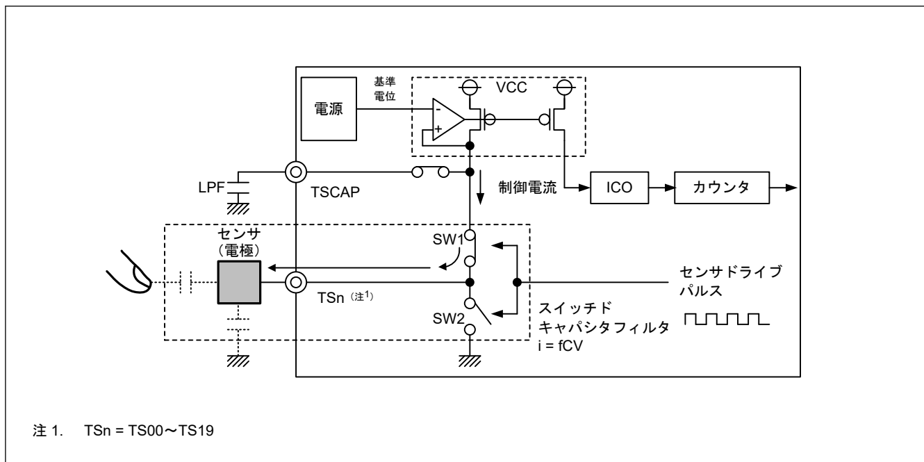
図 46.5 充電動作
