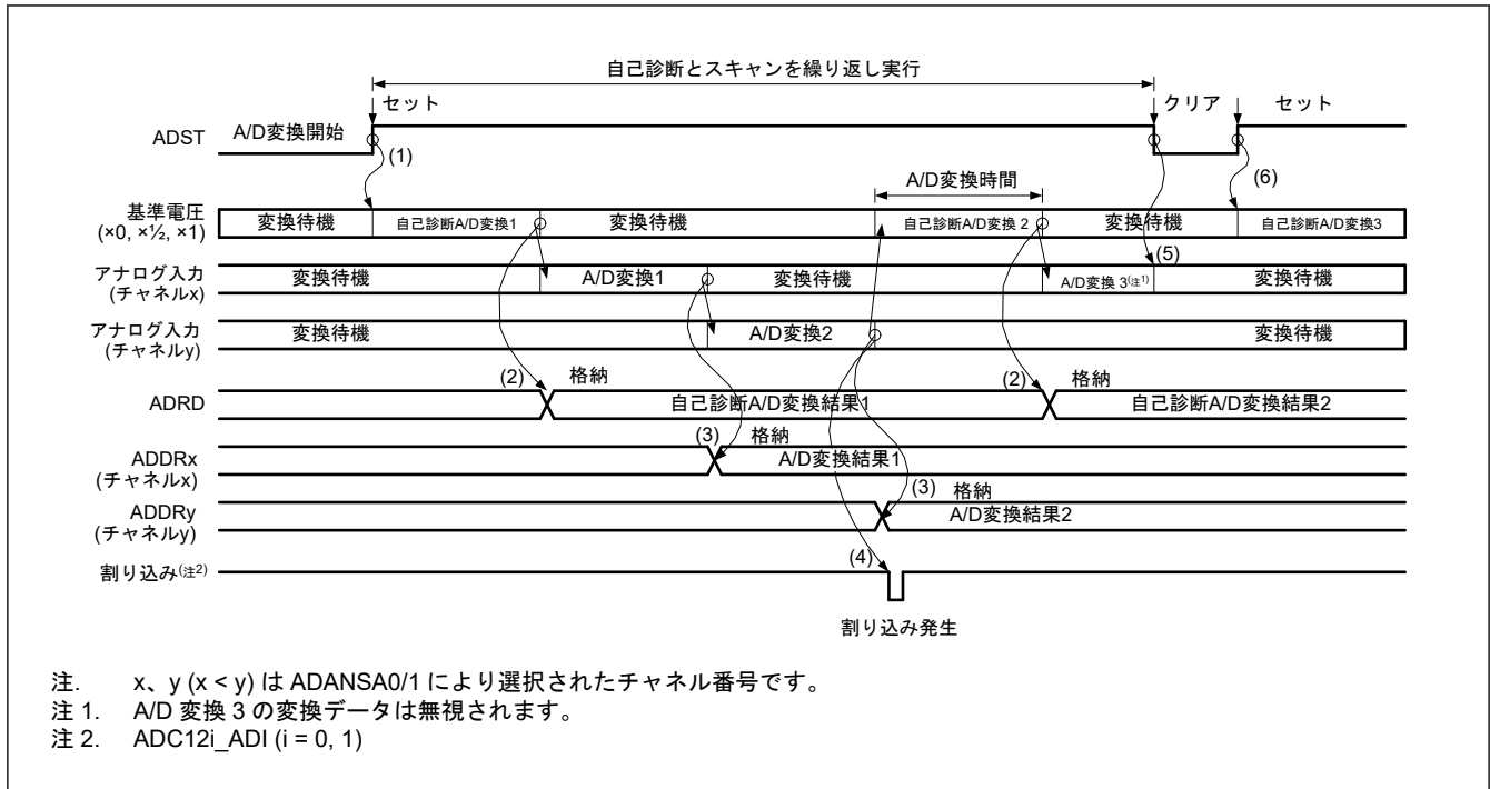
図 43.14 連続スキャンモードの基本動作例 (アナログ入力 (チャンネル x, y) 選択+自己診断)
