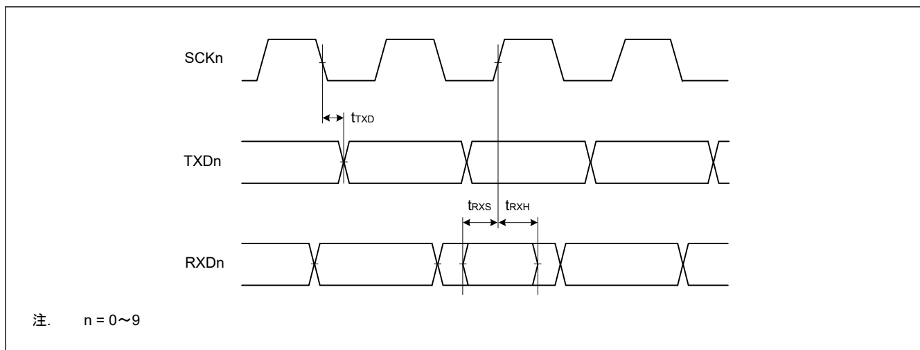
図 53.35 クロック同期式モードにおける SCI 入出力タイミング
