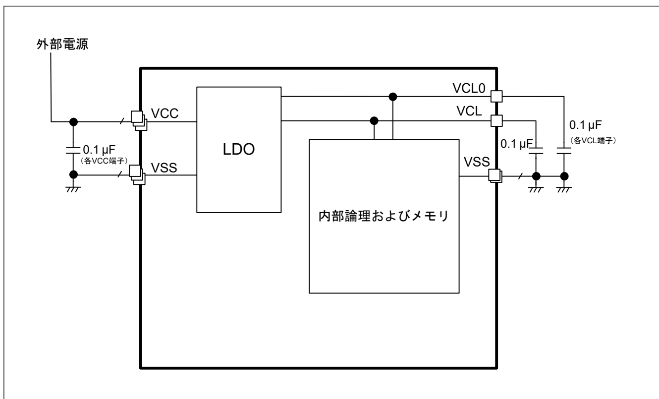
図 51.1 LDO モード設定
