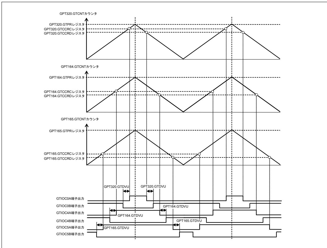
図 21.44 非対称三角波 3 相相補 PWM 出力例 (デッドタイム自動設定)
