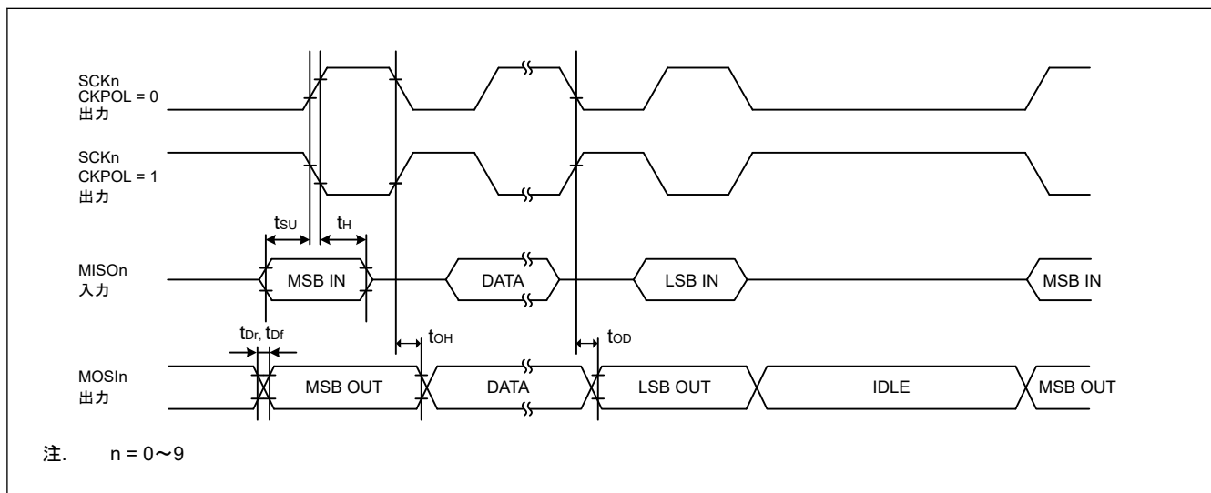
図 53.37 CKPH = 1 の場合におけるマスタの SCI 簡易 SPI モードタイミング
