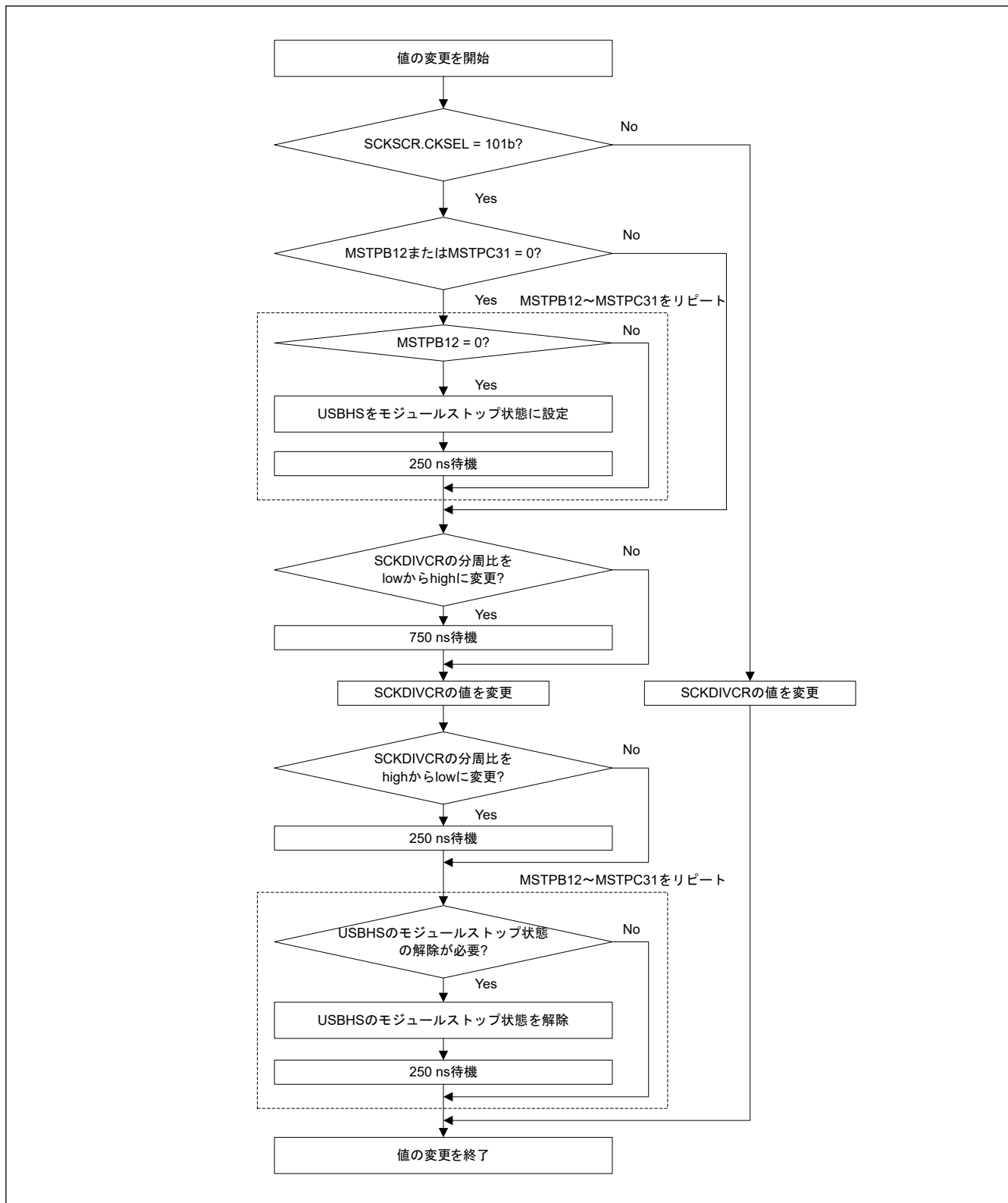
図 8.2 SCKDIVCR の値の変更フロー例
