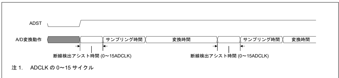
図 43.33 断線検出アシスト機能を使用した場合の A/D 変換動作図
