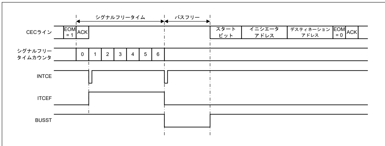
図 37.46 シグナルフリータイムの動作
