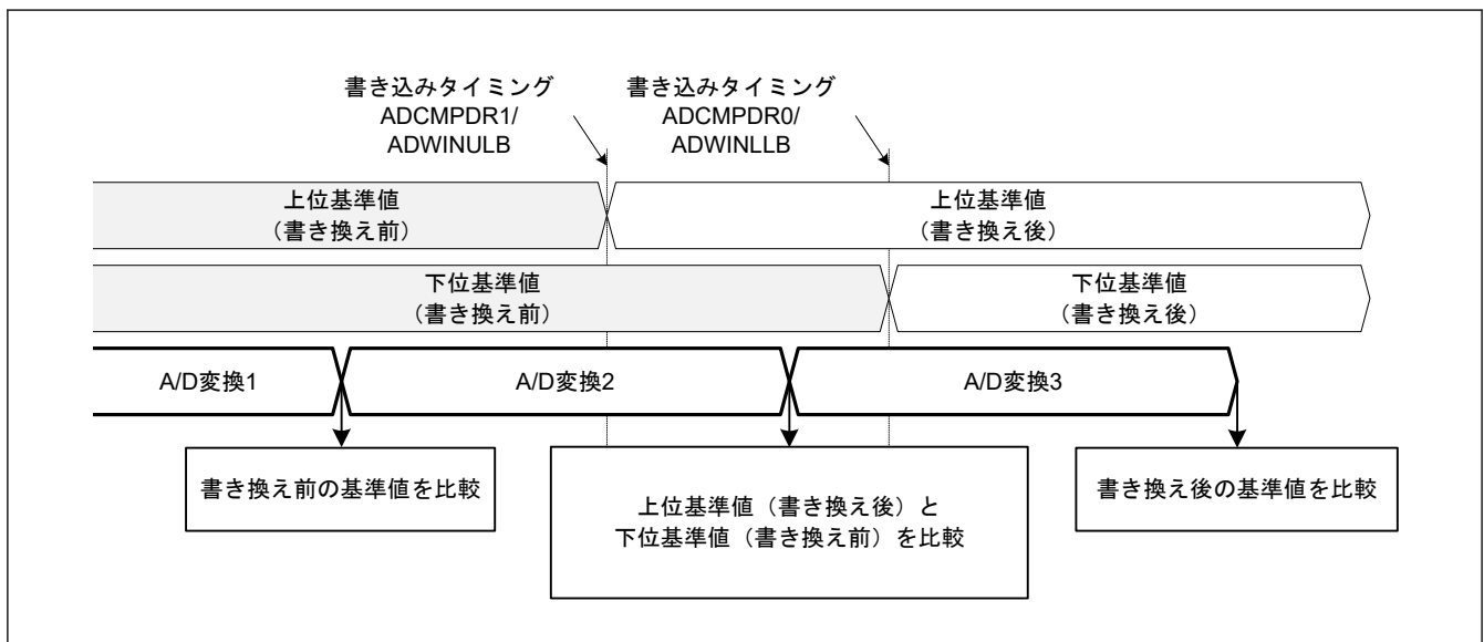
図 43.6 書き換え前後の上側基準値と下側基準値の比較
