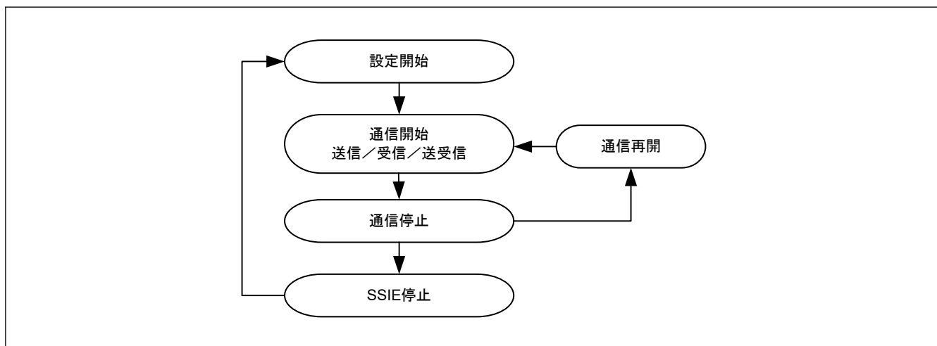
図 38.52 SSIE の通信動作
