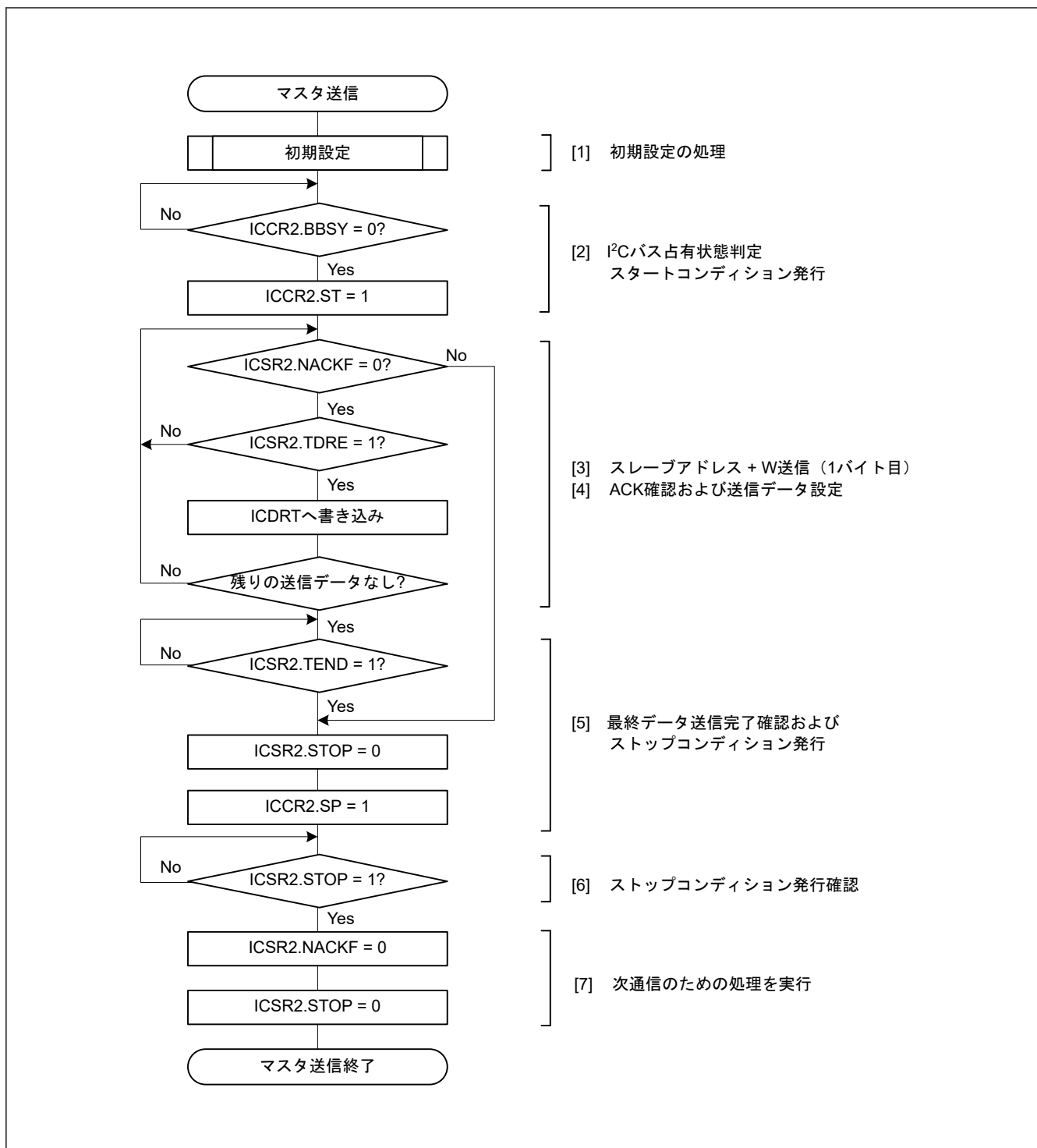
図 31.6 マスタ送信のフローチャート例
