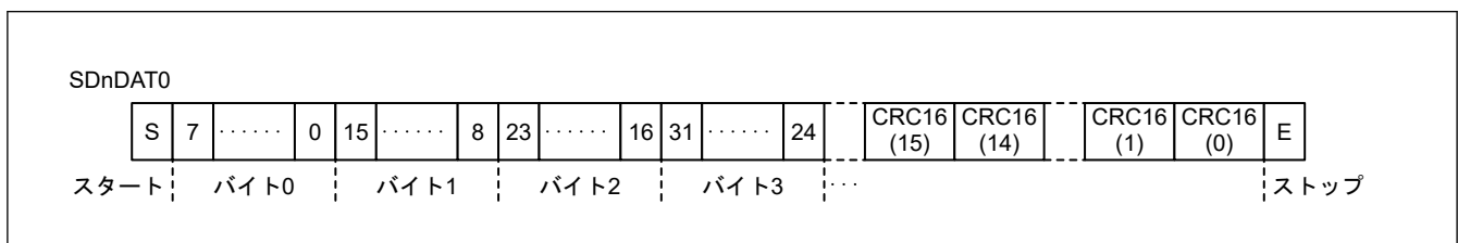
図 39.2 1 ビット幅モードの SDnDAT
