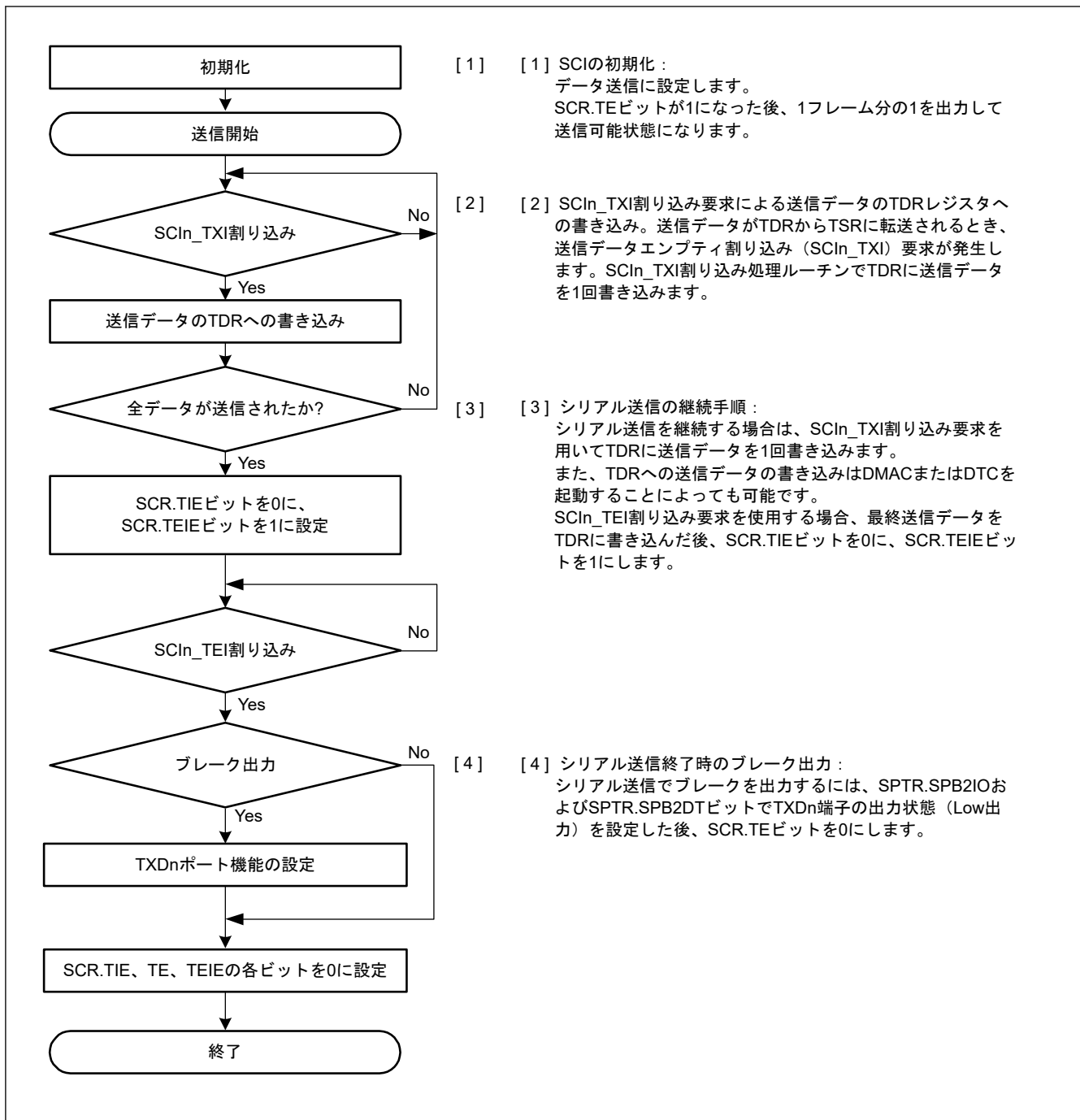
図 30.15 調歩同期式モードにおけるシリアル送信のフローチャート例 (非 FIFO 選択時)
