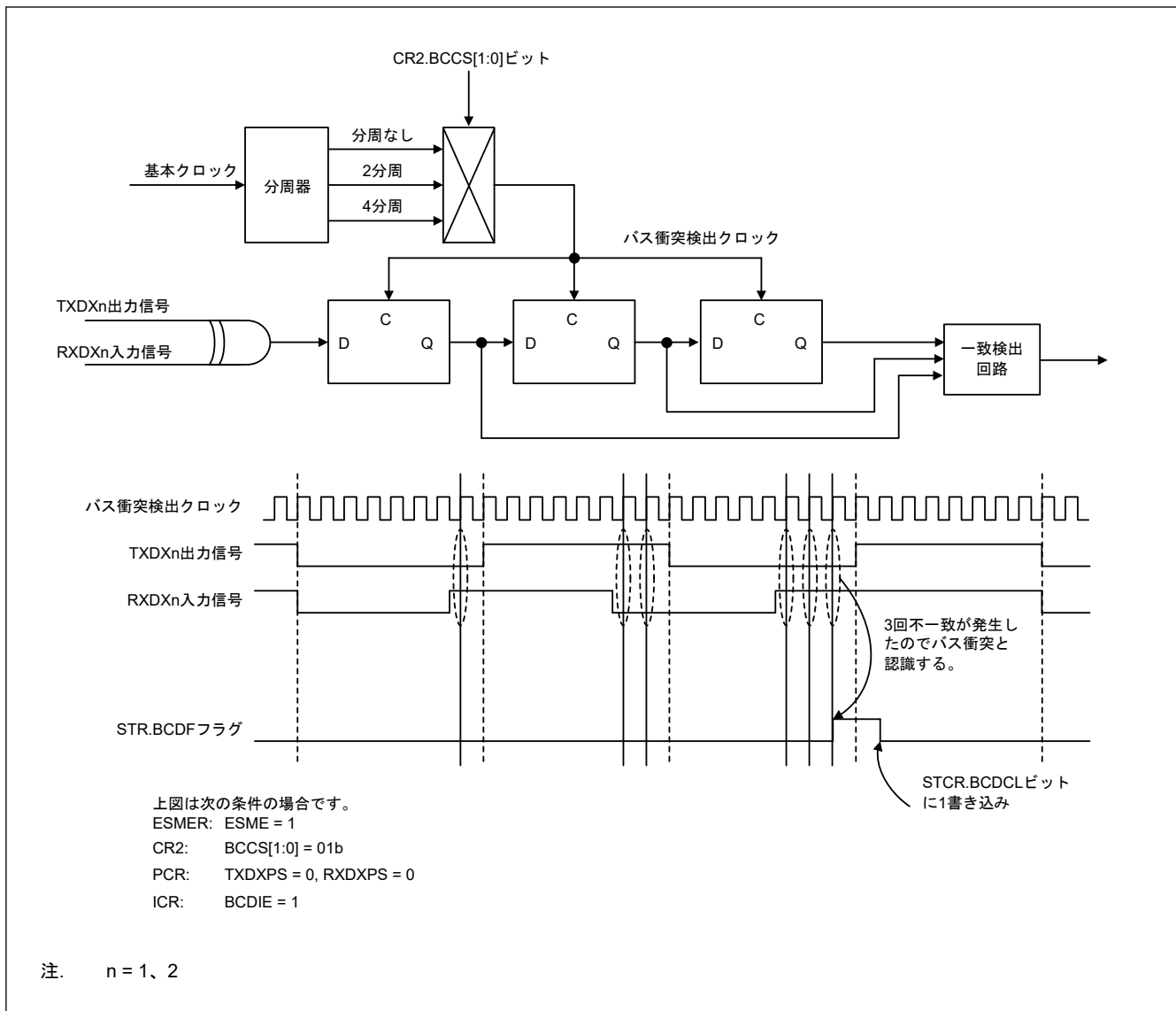
図 30.111 バス衝突検出機能の動作例
