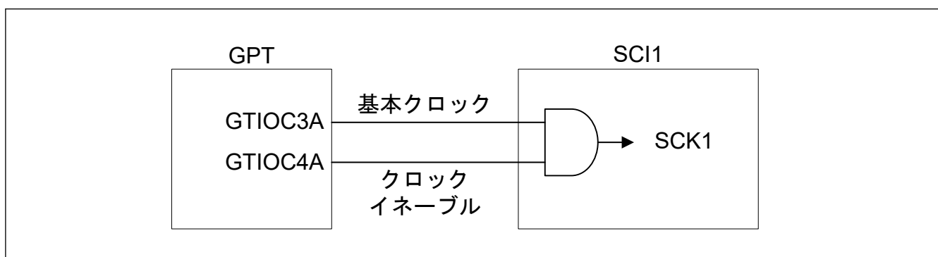
図 30.3 GPT と SCI の接続例
