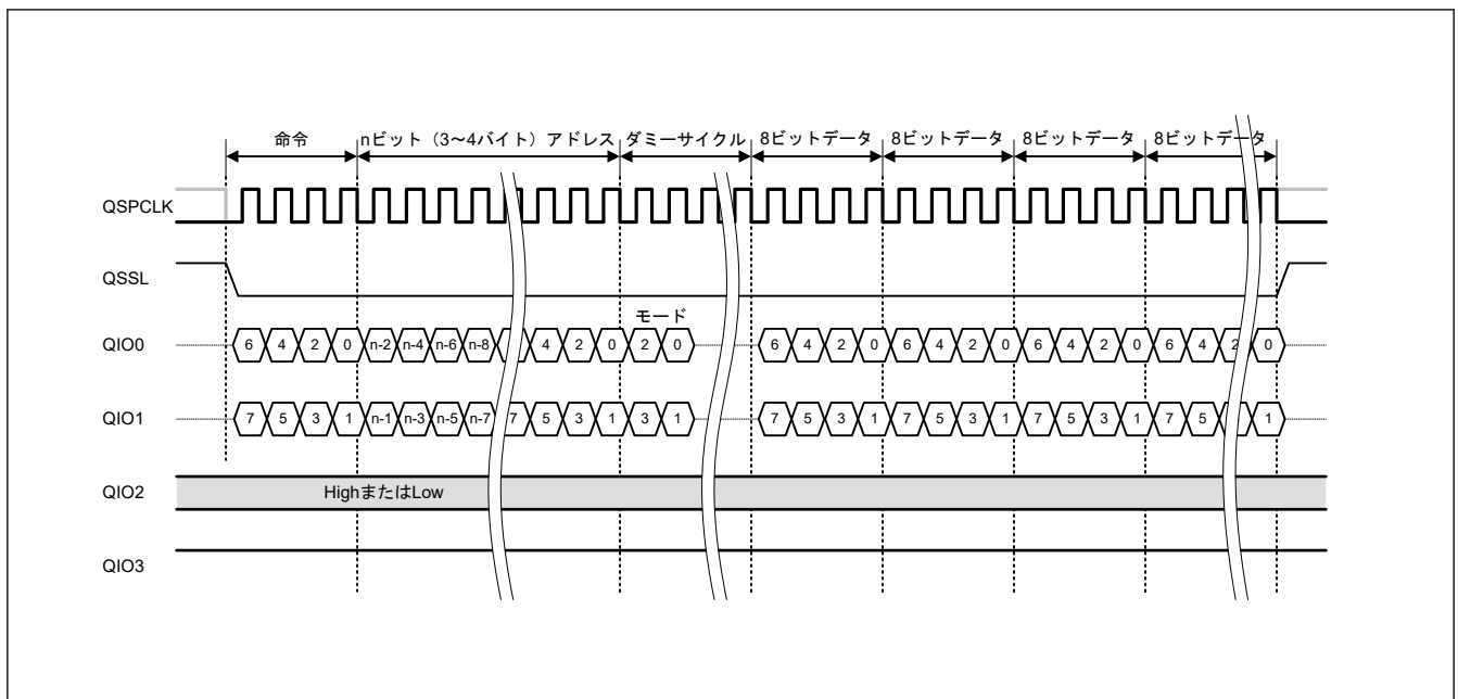
図 35.6 Dual-SPI プロトコル例 (ファストリード Dual I/O)
