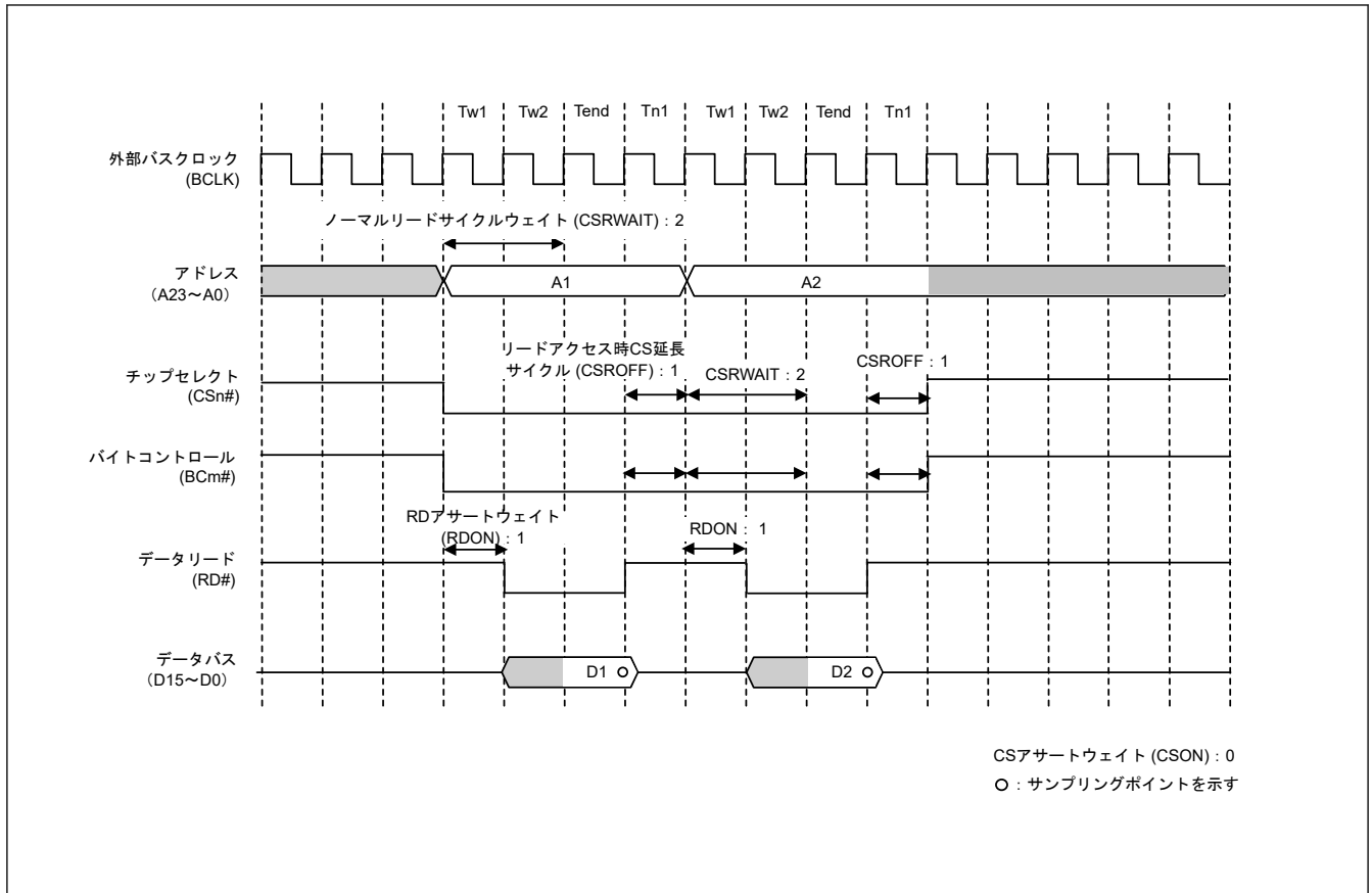
図 14.10 ノーマルリードアクセスの動作例 (1 転送要求に対して 2 回バスアクセスが発生する場合) (n = 0~7、m = 0~1)
