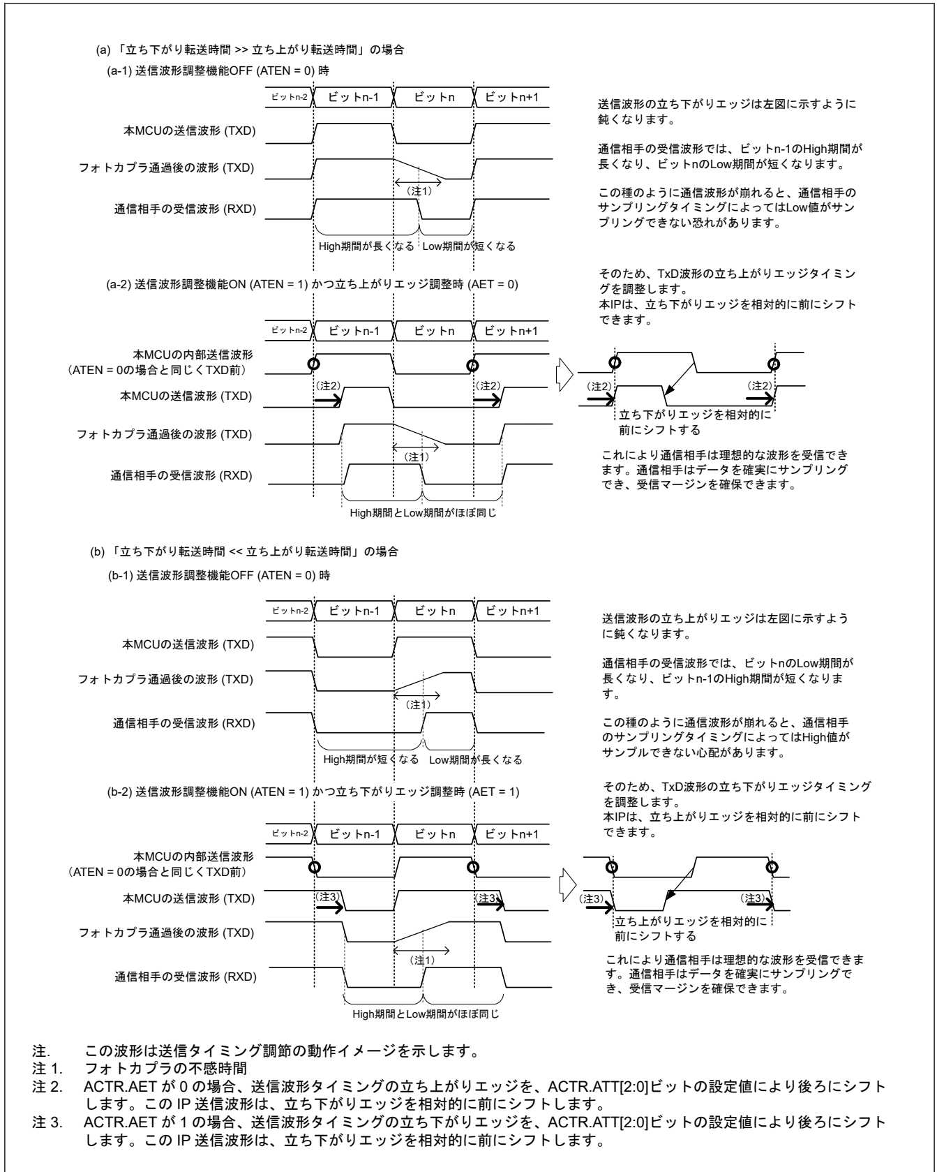
図 30.36 フォトカプラを通過する通信の送信動作の概要
