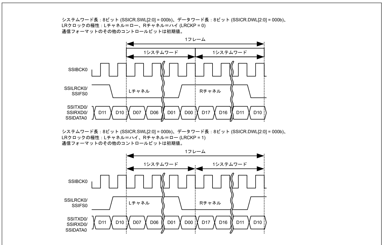
図 38.12 LR クロック/フレーム同期極性設定
