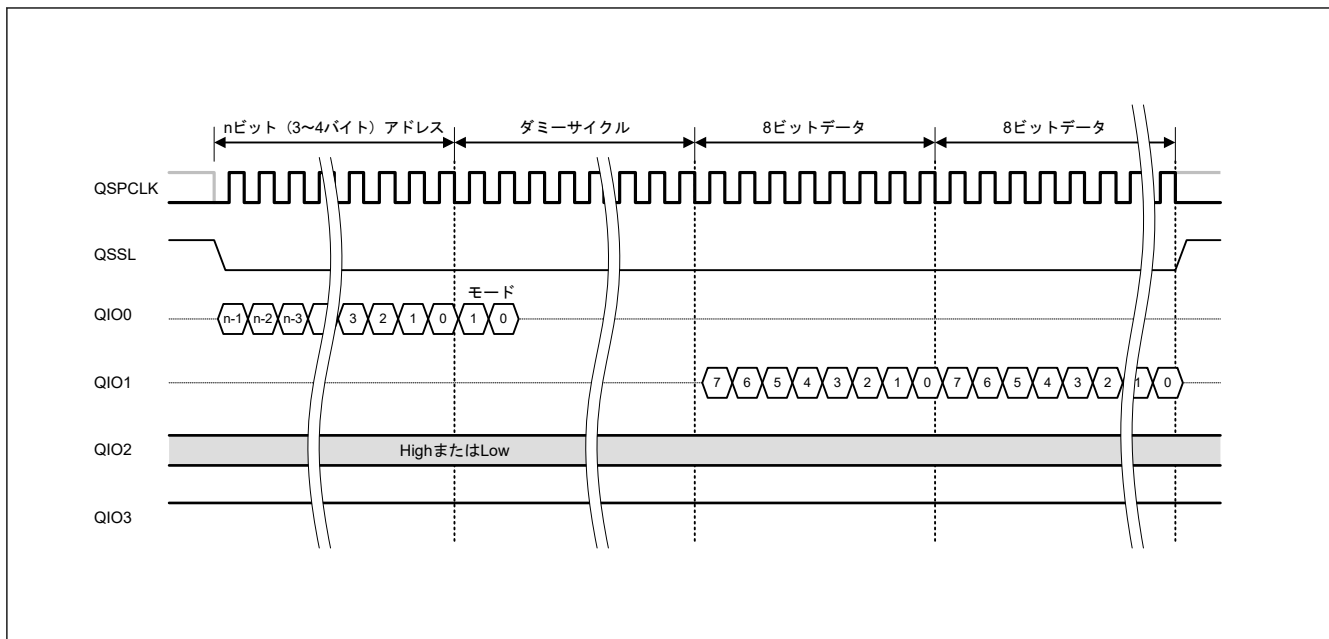
図 35.20 XIP モード時のファストリードバスサイクル
