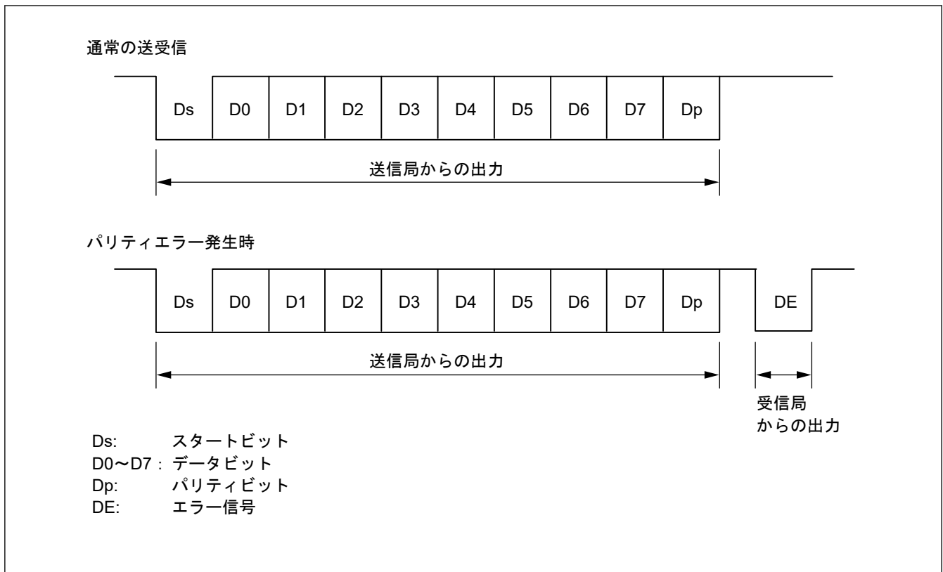
図 30.78 スマートカードインタフェースモードにおけるデータフォーマット
