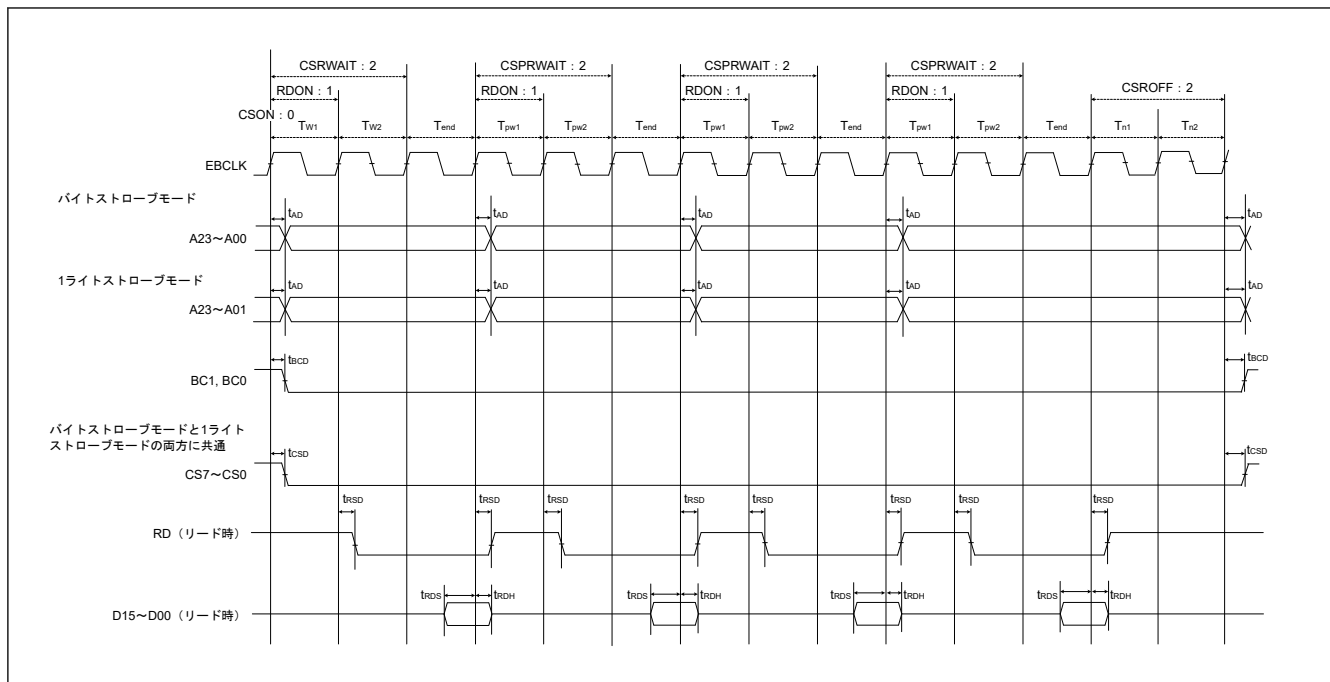
図 53.24 バスクロック同期を使用したページリードサイクルの外部バスタイミング
