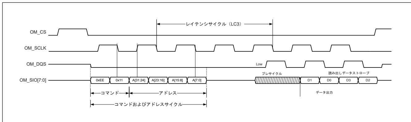
図 36.10 OctaRAM インタフェースでの読み出し動作の波形 (プレサイクル許可を使用した DOPI モード)
