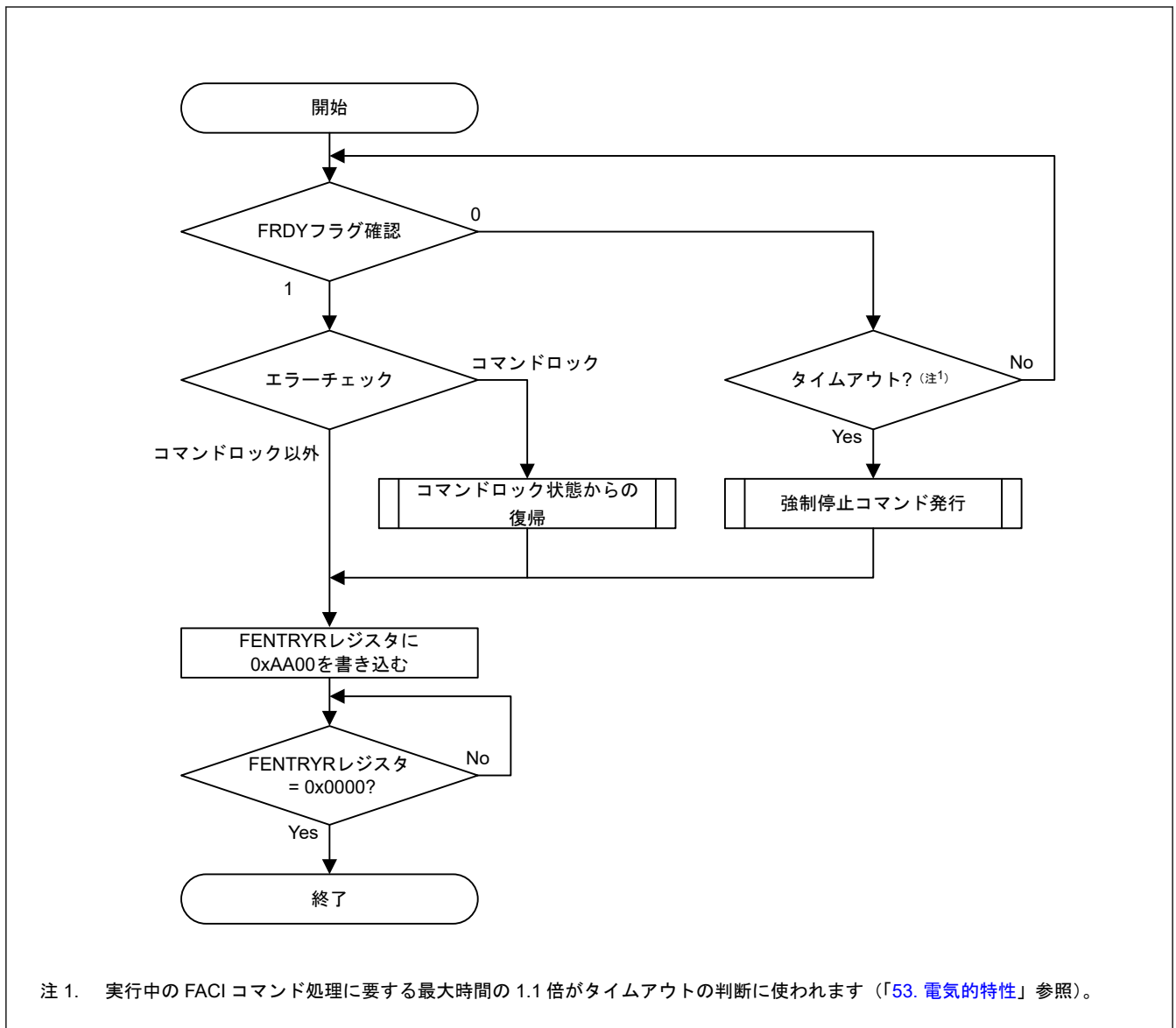
図 50.12 読み出しモードへの遷移手順
