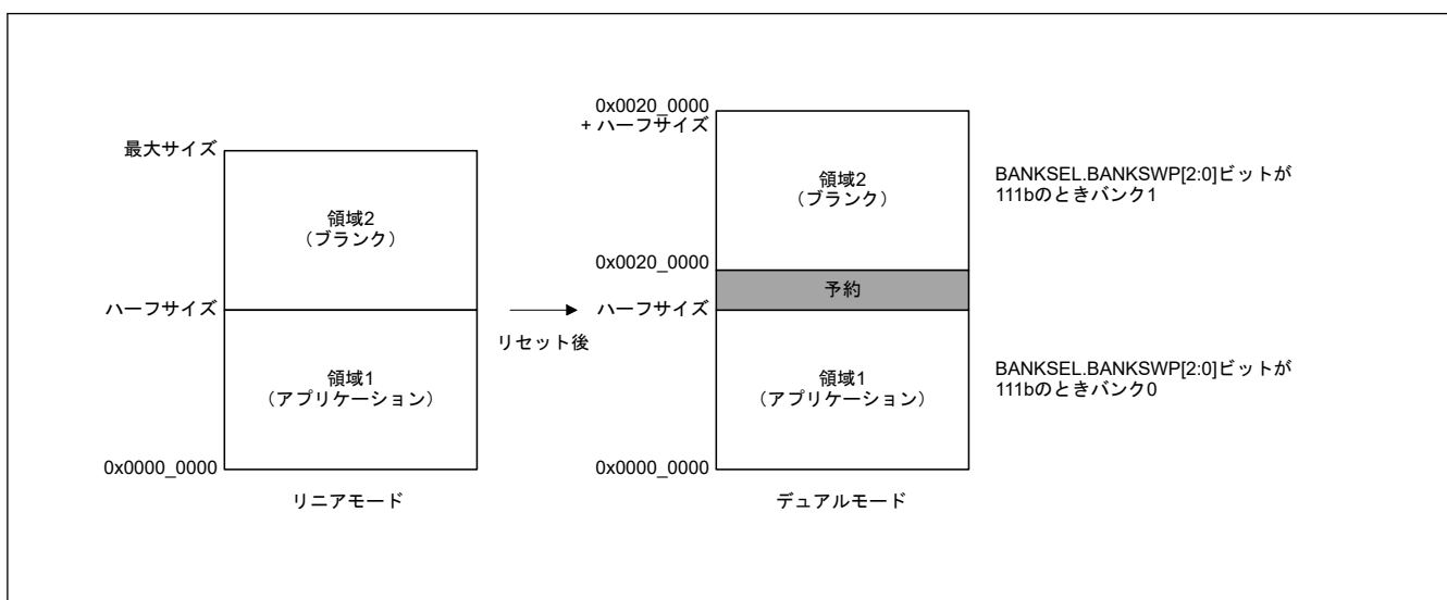
図 50.47 リニアモードでのデュアルモード用アプリケーションの書き込み
