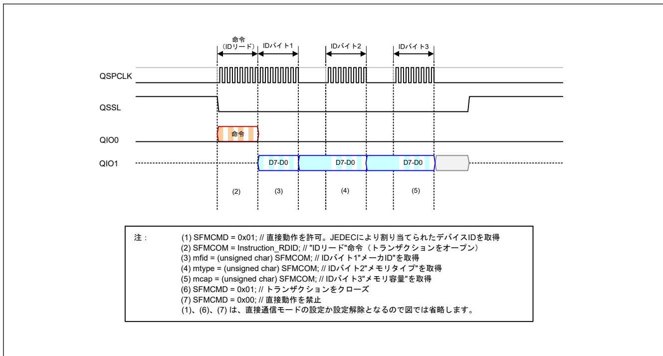
図 35.41 ID リードの直接通信タイミング例
