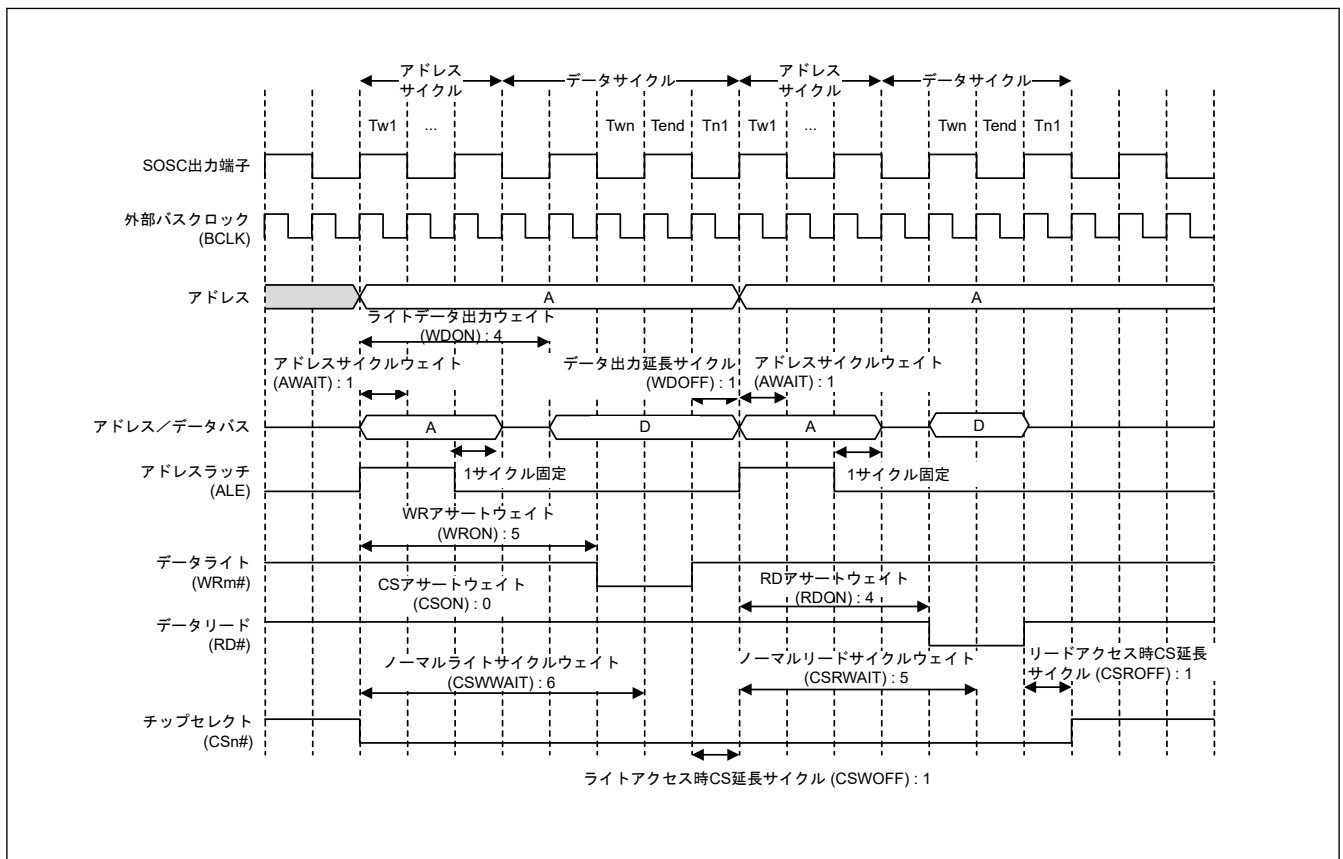
図 14.25 アドレス/データマルチプレクス I/O インタフェース時のバスタイミング例 (m = 0、1)
