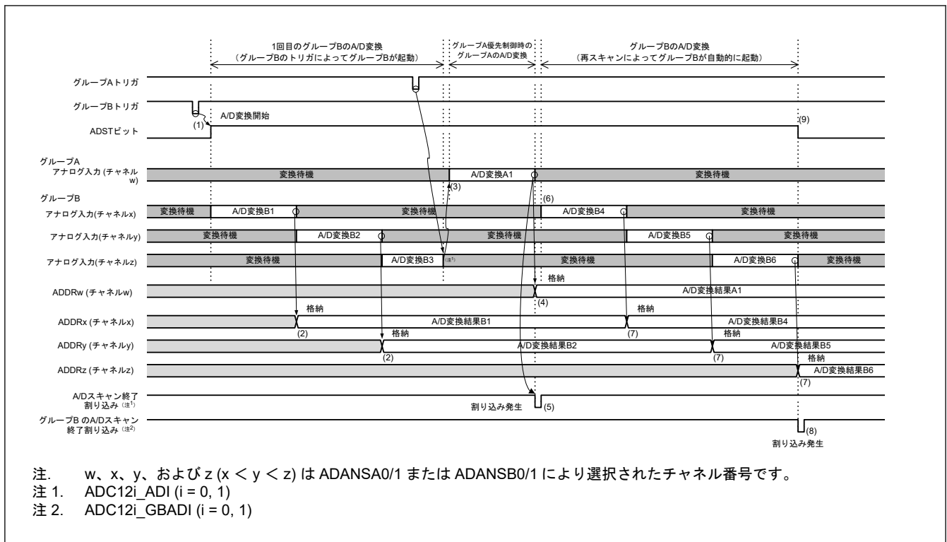
図 43.19 グループ優先動作の例 1-1 : グループ B スキャン中のグループ A トリガ入力、再スキャンあり (ADGSPCR.GBRSCN = 1、ADGSPCR.GBRP = 0、および ADGSPCR.LGRRS = 0 の場合)
