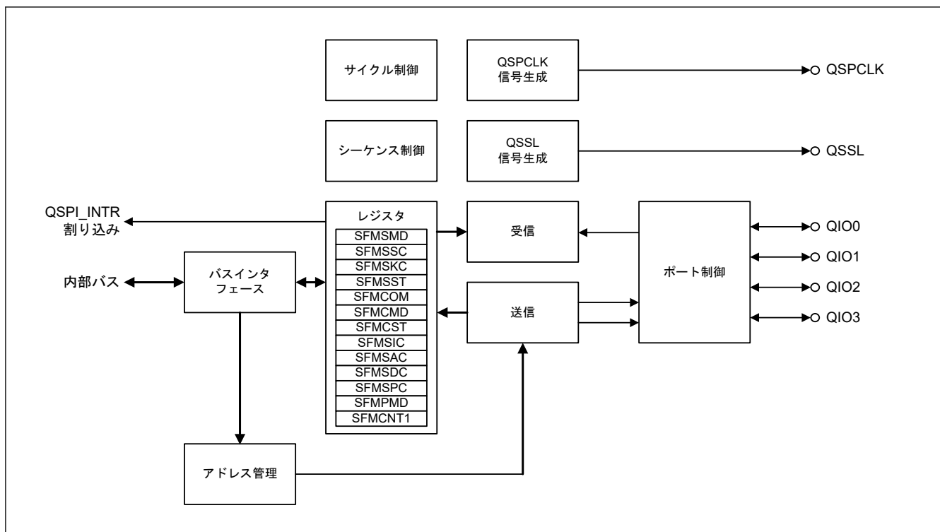
図 35.1 QSPI のブロック図
