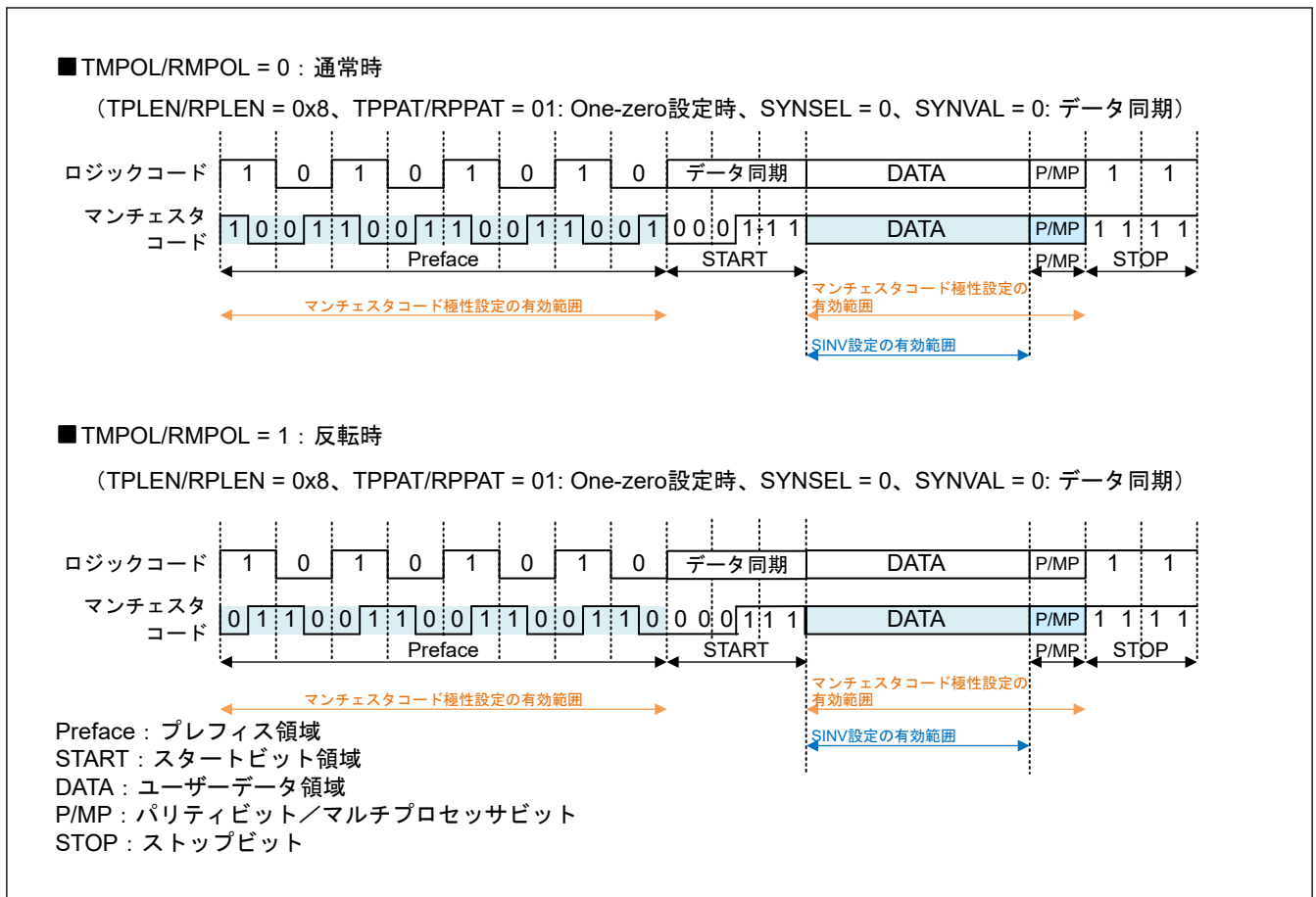
図 30.64 マンチェスタコード極性設定の有効範囲
