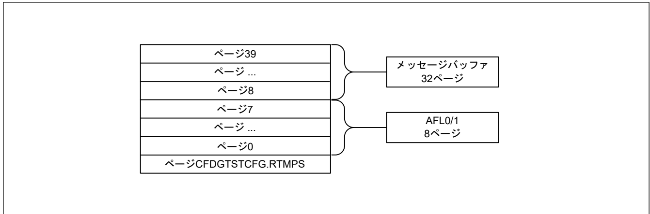
図 32.51 RAM のページ構造
