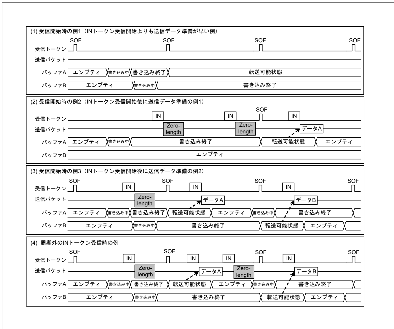
図 29.16 データセットアップ動作例
