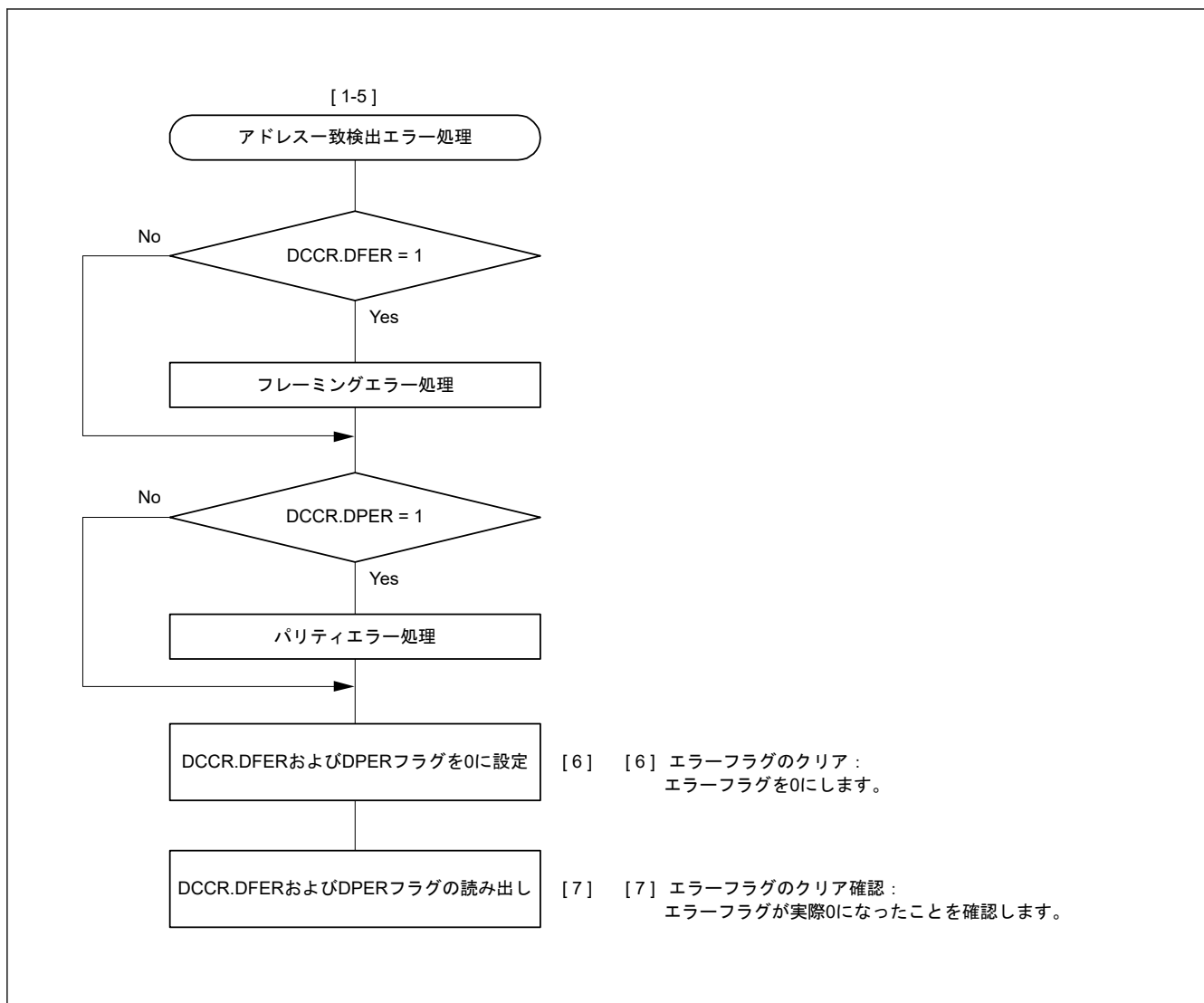
図 30.23 調歩同期式モードにおけるシリアル受信のフローチャート例（非 FIFO 選択、アドレス一致検出有効時）(2)
