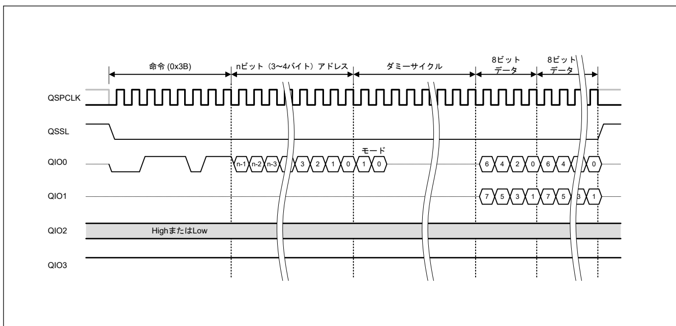
図 35.21 拡張 SPI プロトコルでのファストリード Dual 出力バスサイクル
