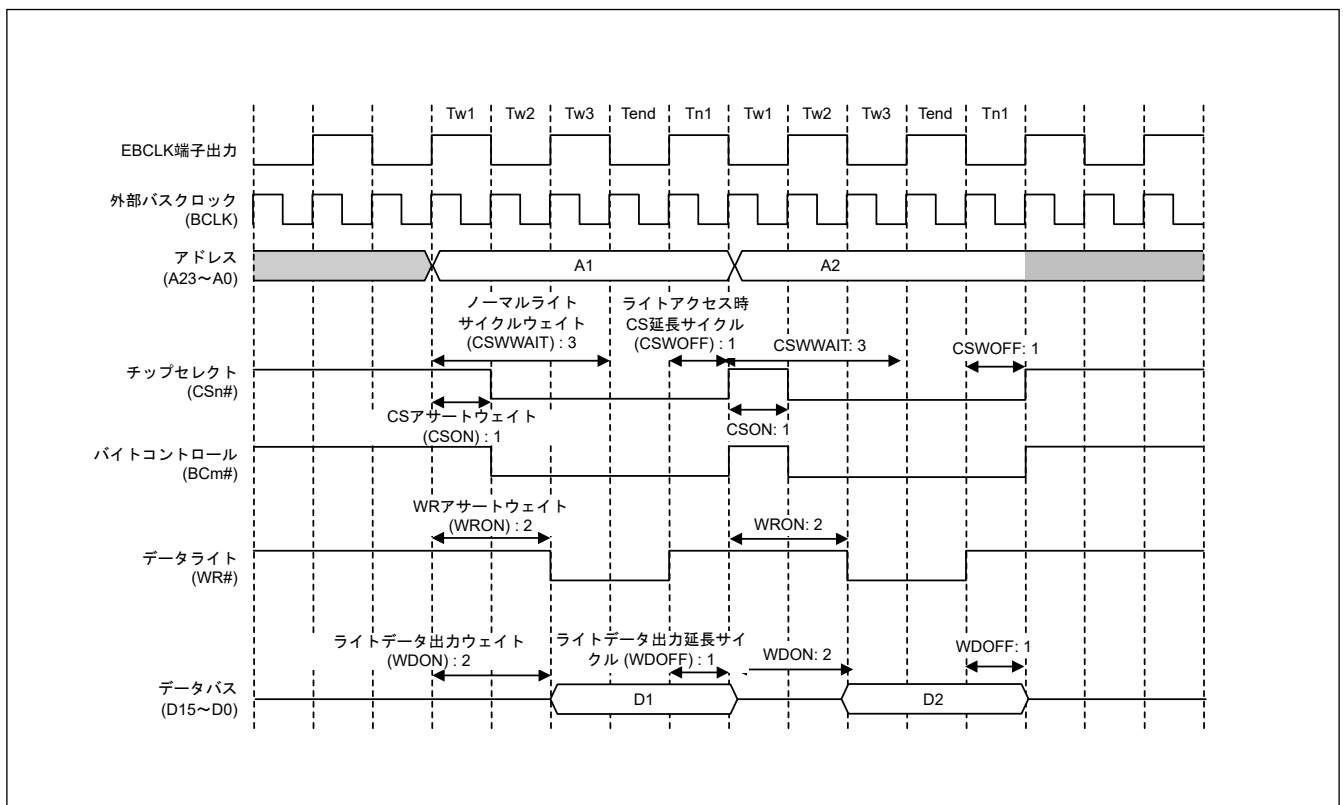
図 14.16 ノーマルライトアクセスの動作例 (EBCLK 端子出力選択ビットで BCLK の 2 分周を設定した場合、および 1 転送要求に対して 2 回バスアクセスが発生する場合) (n = 0~7、m = 0~1)
