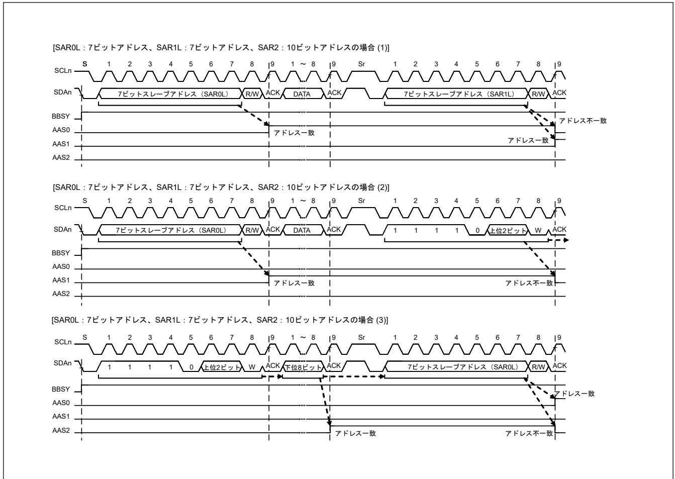
図 31.26 AASn フラグが 1 または 0 になるタイミング (7 ビット/10 ビットアドレスフォーマット混在)
