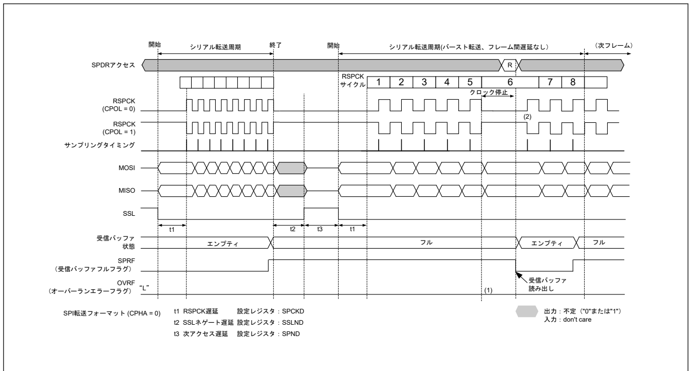
図 34.41 マスタモードの受信バッファフル状態でシリアル転送が継続する場合のクロック停止波形 (バースト転送でフレーム間遅延なし、CPHA = 0)
