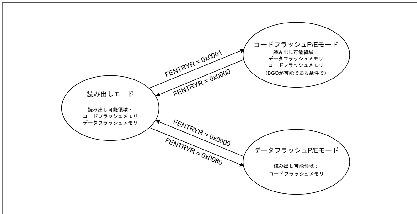
図 50.7 フラッシュシーケンサのモード
