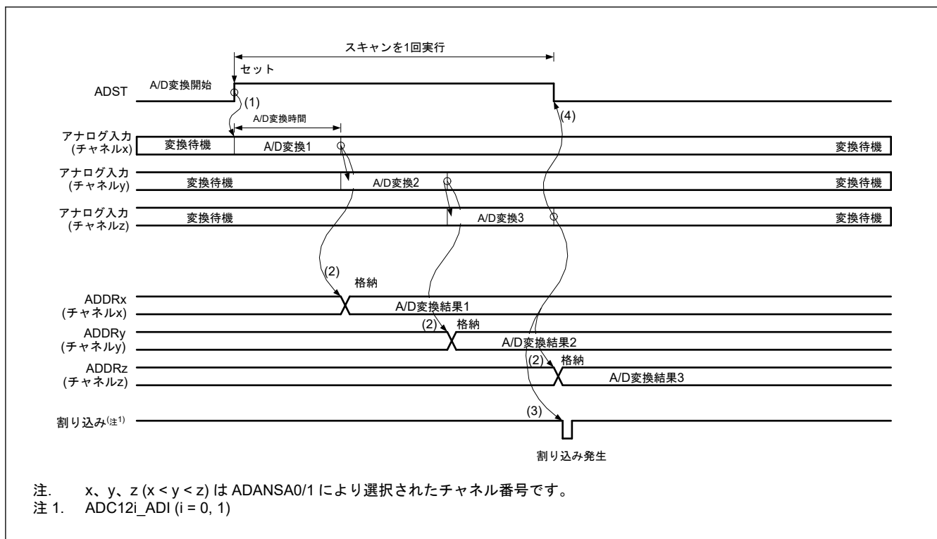
図 43.8 シングルスキャンモードの基本動作例（アナログ入力（チャンネル x~z）選択）
