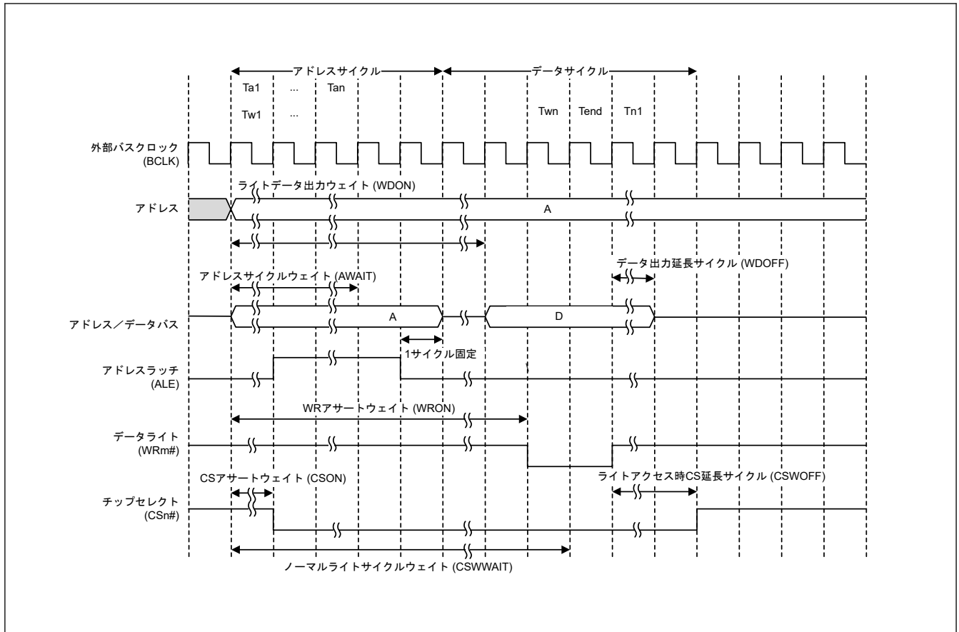
図 14.24 アドレス/データマルチプレクス I/O インタフェース時のライトアクセスの動作例 (m = 0、1)
