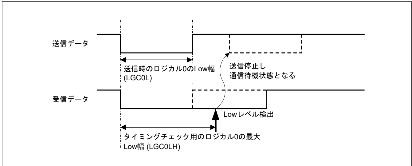
図 37.18 エラー処理パルス受信動作
