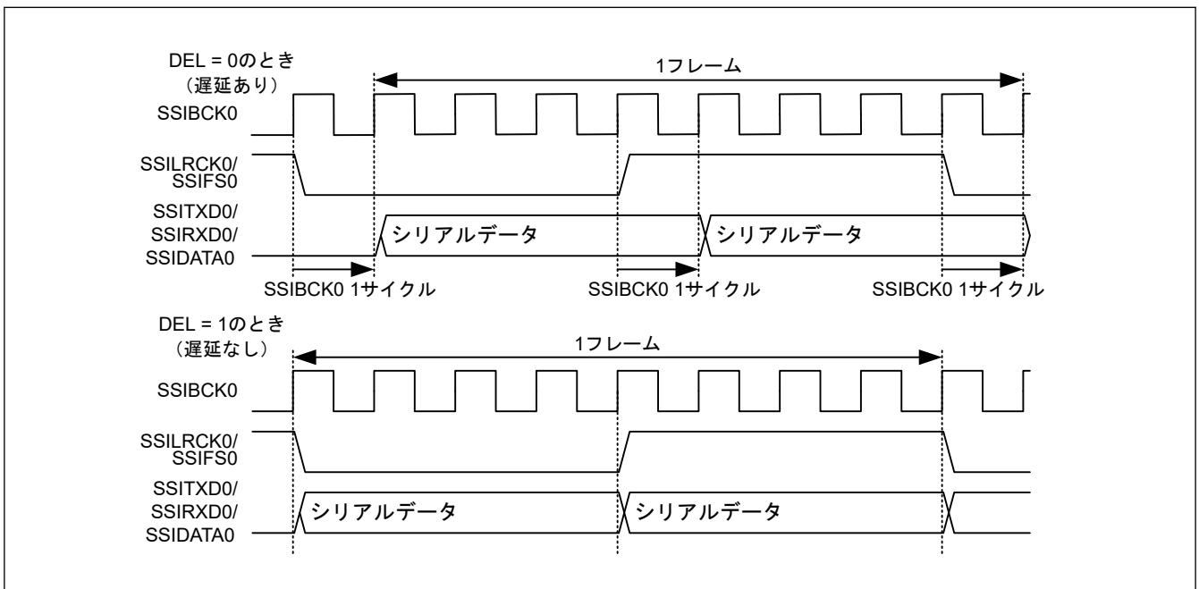
図 38.7 シリアルデータにおける遅延の設定
