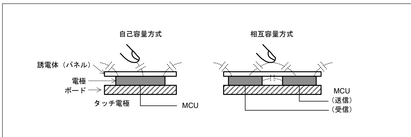
図 46.2 自己容量方式と相互容量方式
