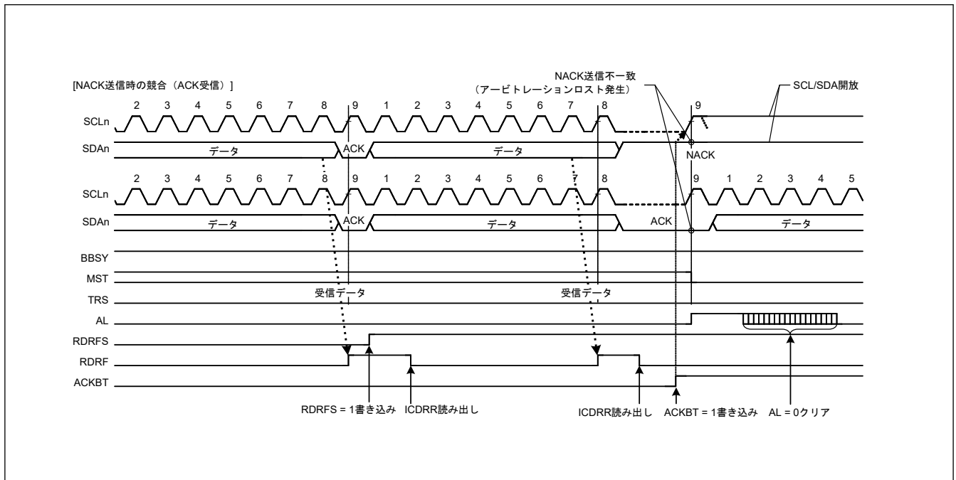
図 31.43 NACK 送信中のアービトレーションロスト検出の動作例 (NALE = 1 の場合)
