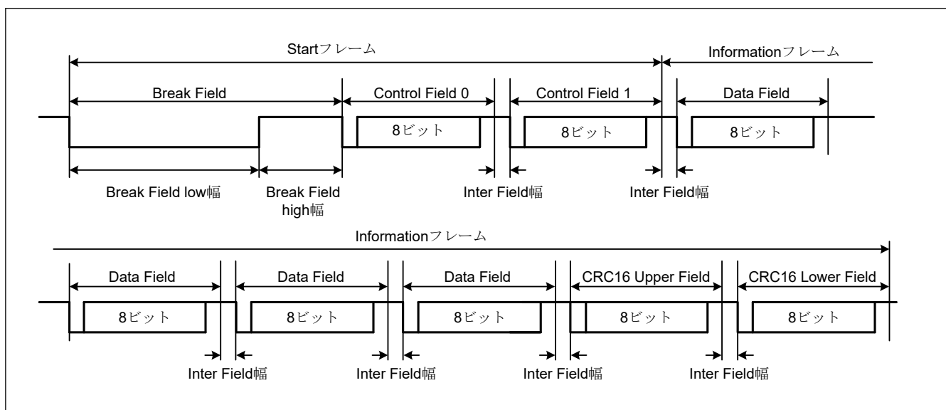
図 30.101 拡張シリアルモード制御部シリアル通信プロトコル
