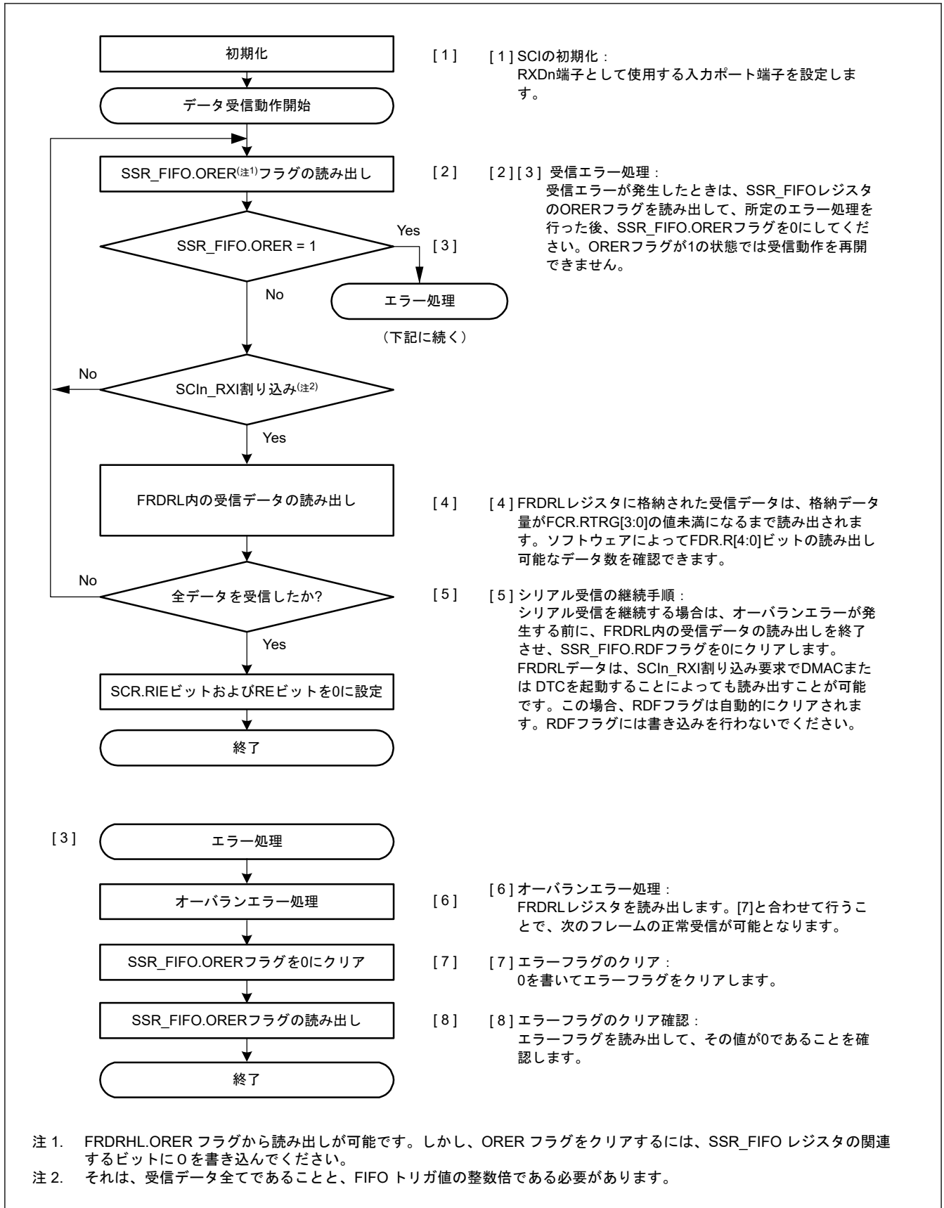
図 30.74 クロック同期式モードにおけるシリアル受信のフローチャート例 (FIFO 選択時)
