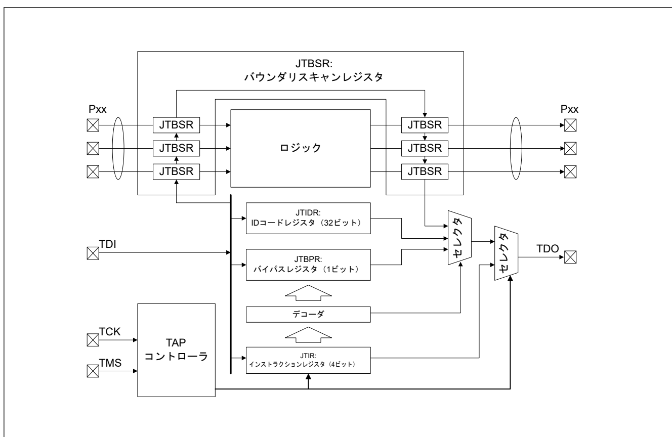
図 41.1 バウンダリスキャン機能のブロック図
