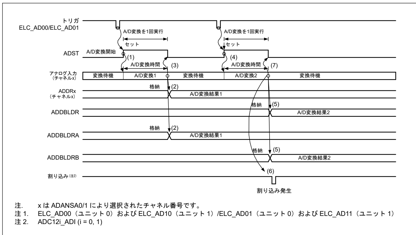
図 43.12 アナログ入力 (チャンネル x) と ELC_AD00 (ユニット 0) および ELC_AD10 (ユニット 1) /ELC_AD01 (ユニット 0) および ELC_AD11 (ユニット 1) の重複選択時のダブルトリガモード拡張動作例
