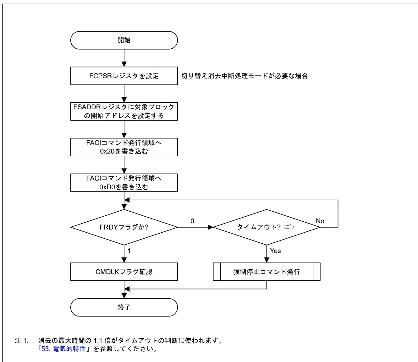
図 50.15 ブロックイレースコマンドの使用フロー
