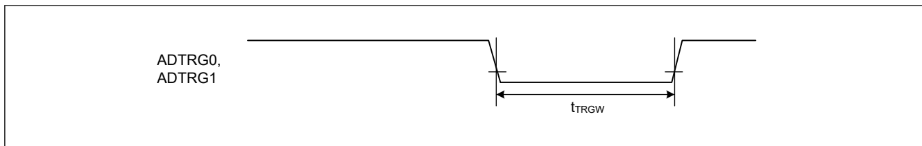
図 53.33 ADC12 トリガ入力タイミング
