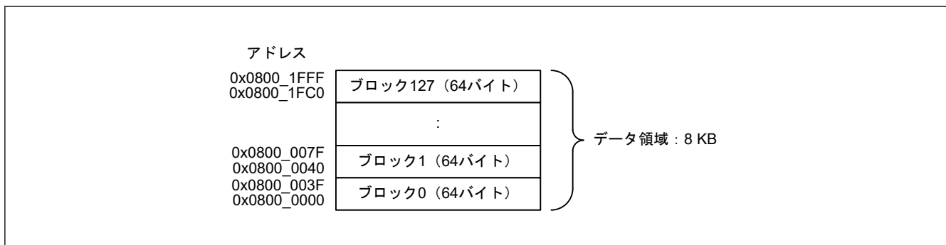
図 50.4 データフラッシュメモリのマップ
