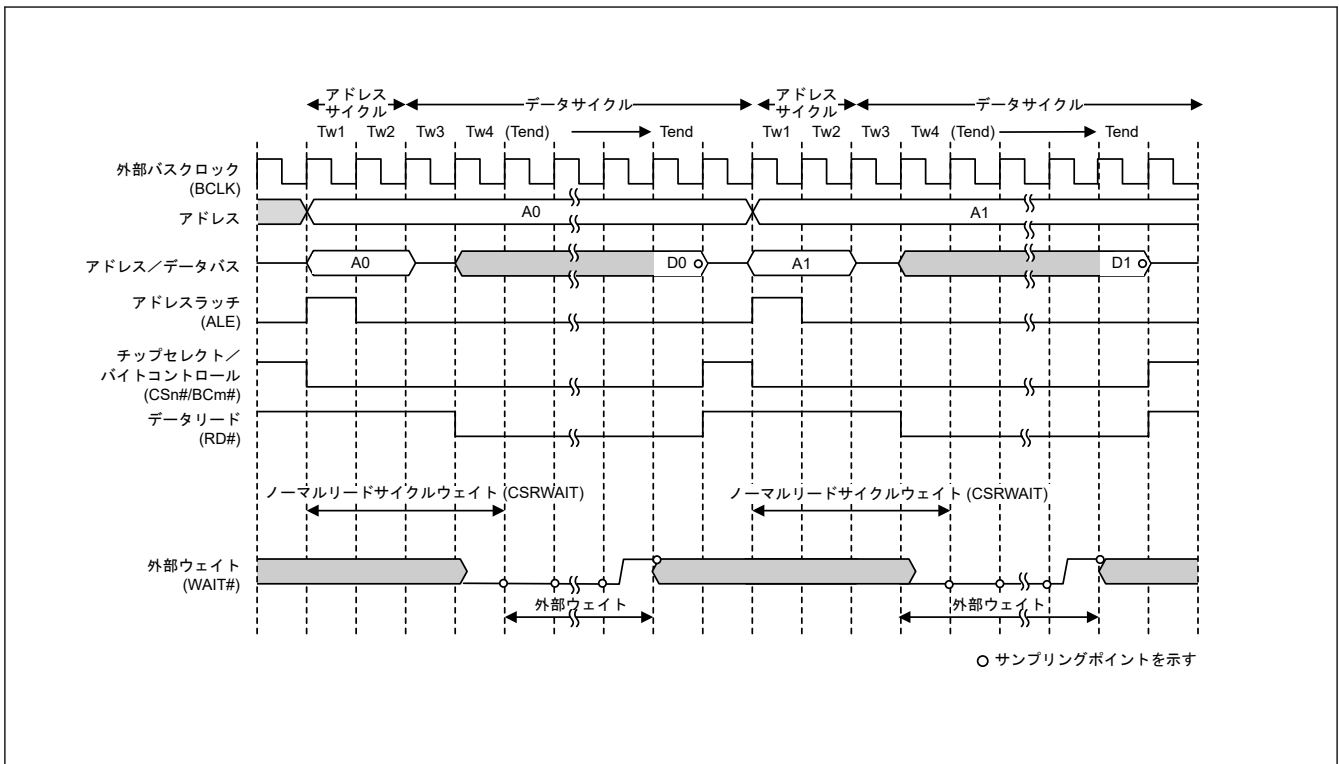
図 14.30 アドレス/データマルチプレクス I/O インタフェース時の外部ウェイト挿入のタイミング例 (m = 0, 1)
