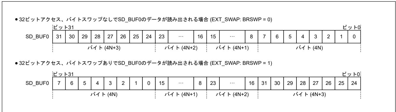
図 39.6 SD_BUF0 からの読み出し
