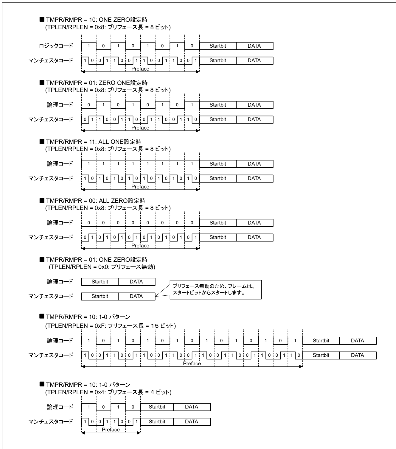
図 30.51 プレフィスパターンの設定例
