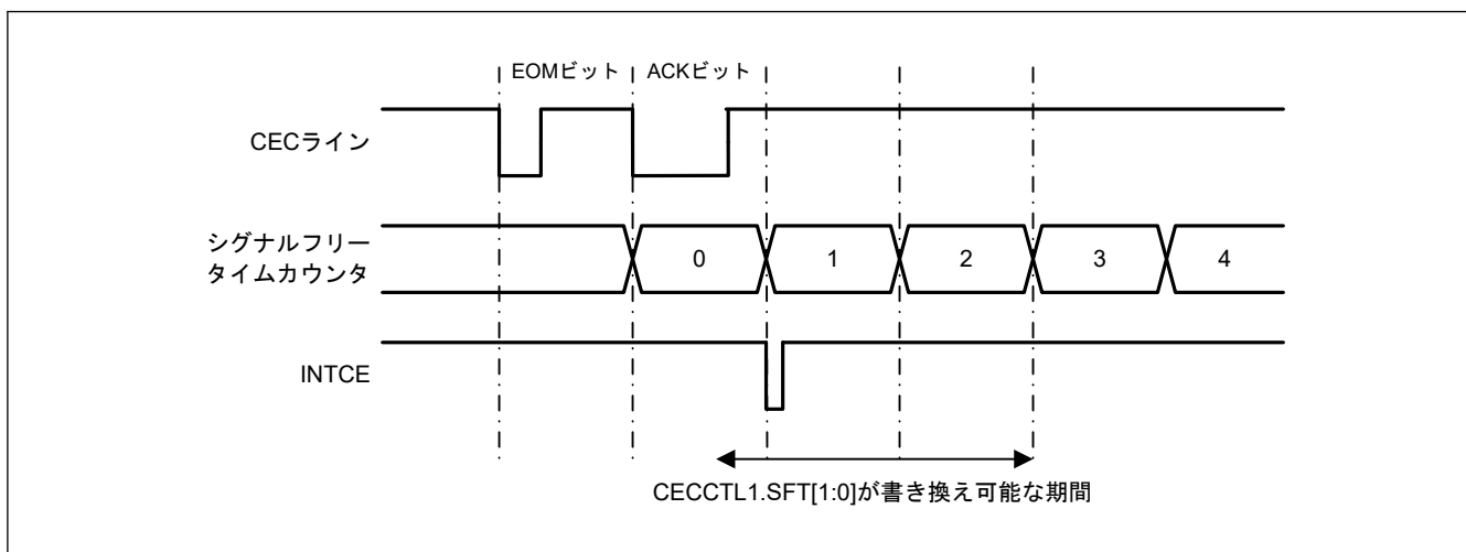
図 37.47 シグナルフリータイムカウント中の CECCTL1.SFT[1:0] ビット書き換え有効期間
