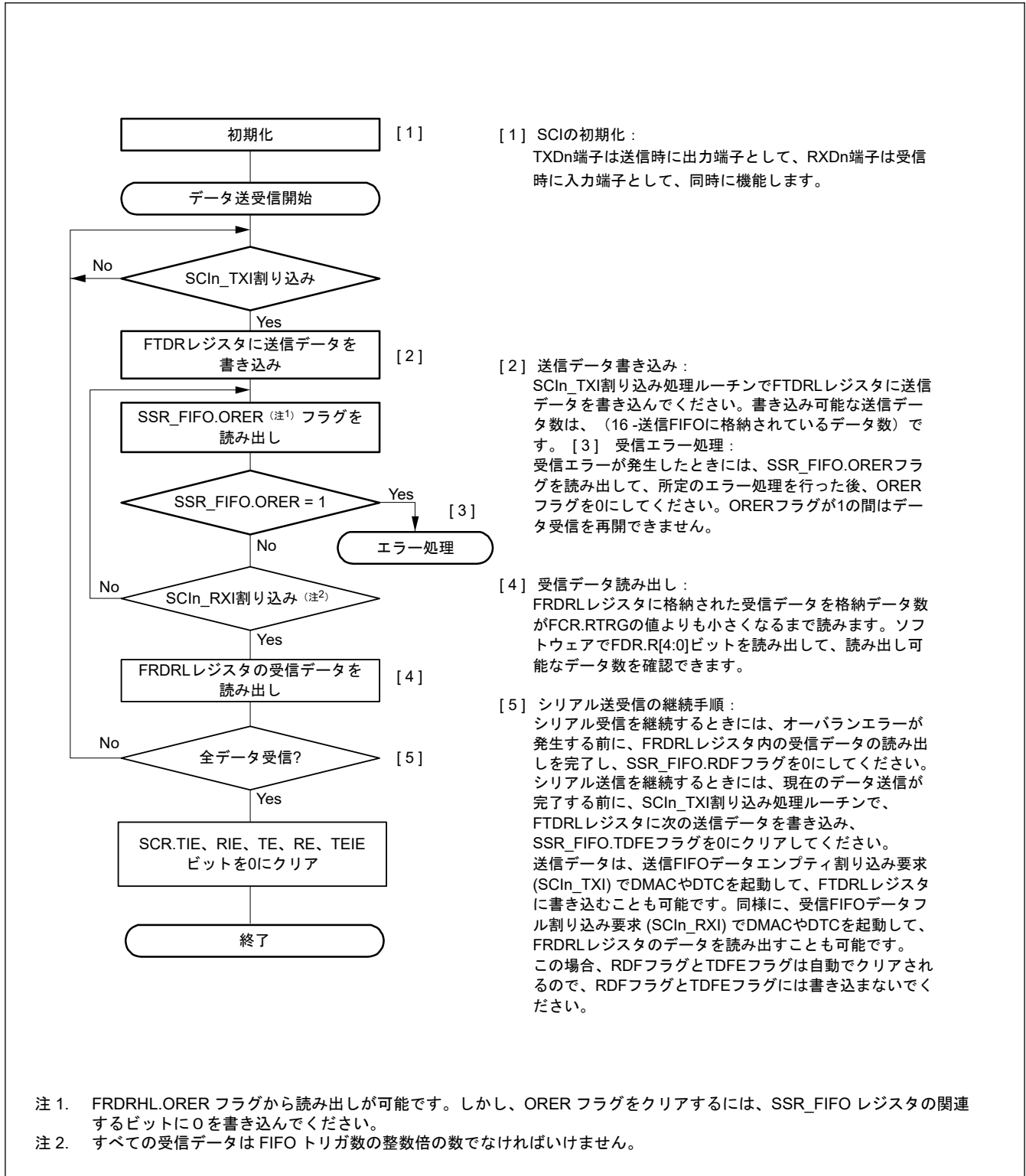
図 30.76 クロック同期式モードにおけるシリアル同時送受信動作のフローチャート例 (FIFO 選択時)
