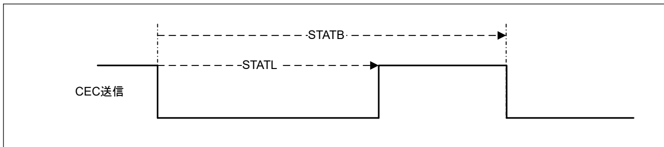
図 37.9 スタートビットの出力波形
