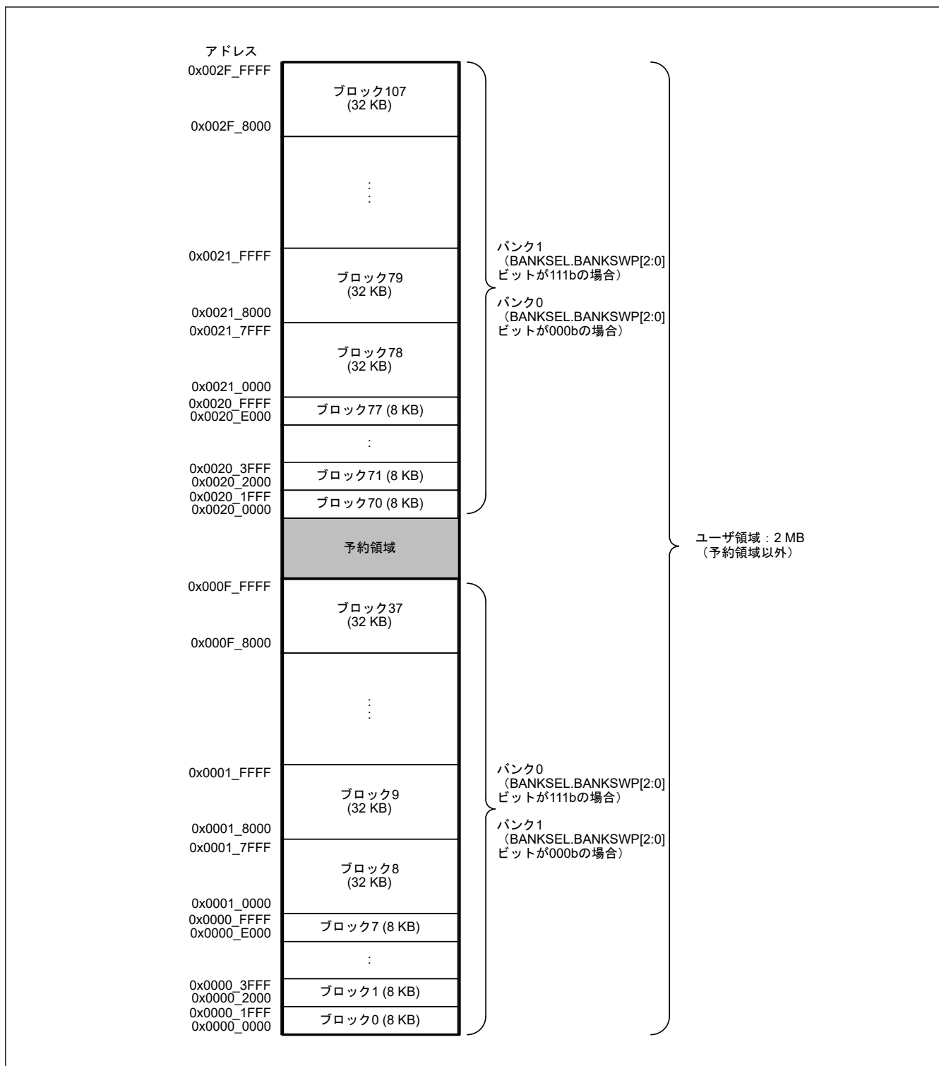
図 50.3 デュアルモードでのコードフラッシュメモリのマップ
