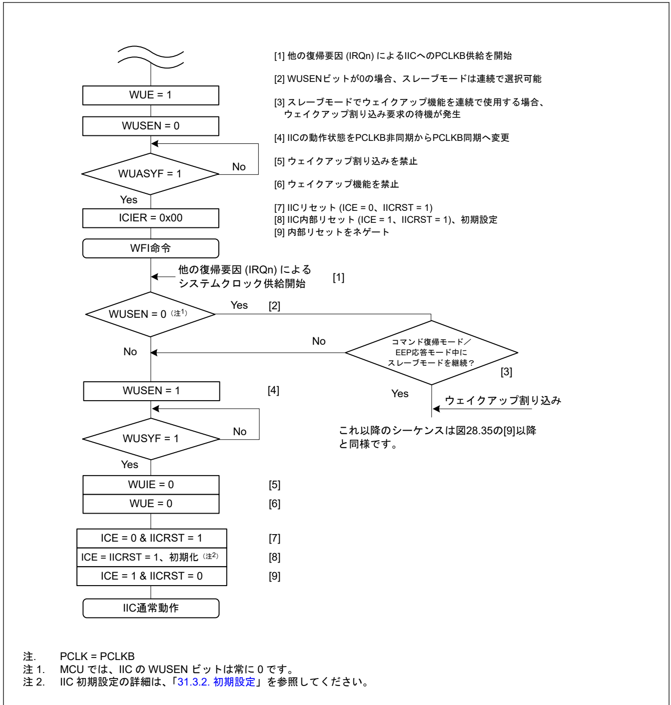
図 31.36 コマンドリカバリモードとEEP 応答モードの動作例 (IIC ウェイクアップ割り込み以外の割り込み (たとえば IRQn) によるウェイクアップの場合)
