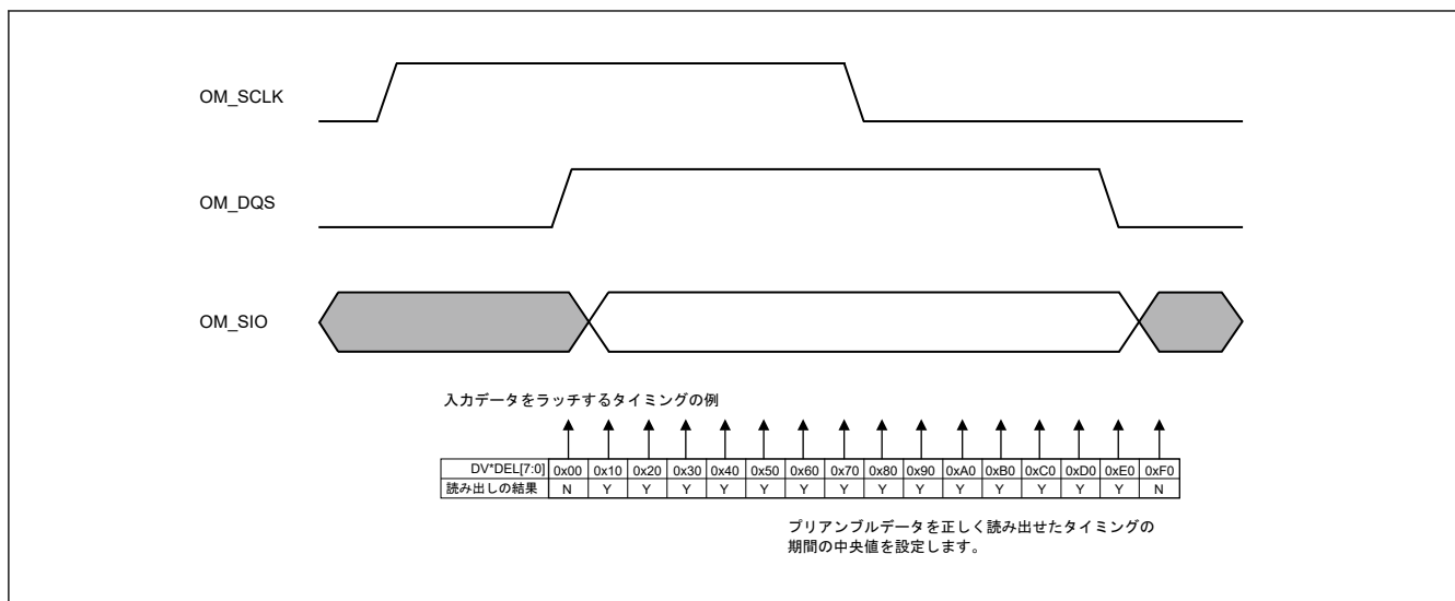
図 36.16 MDTR レジスタの DV0DEL ビットと DV1DEL ビットの初期設定の例
