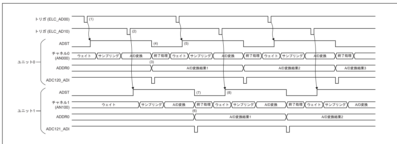
図 43.26 シングルスキャンモードの動作例 (AN000 および AN100 選択、インターリーブ動作)
