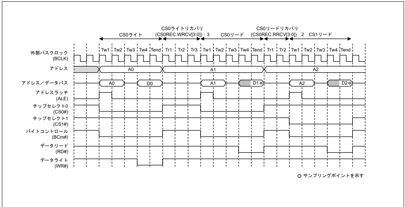
図 14.35 リカバリサイクルの動作例（アドレス／データマルチプレクス I/O インタフェースの場合）(m = 0、1)
