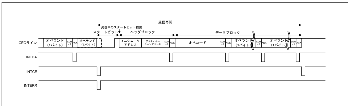
図 37.49 再受信機能動作
