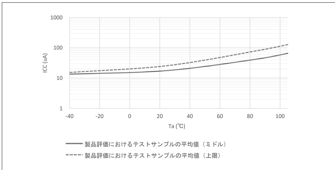
図 53.3 ディープソフトウェアスタンバイモード時の温度依存性、スタンバイ SRAM および USB レジューム検出部への電源供給あり (参考データ)
