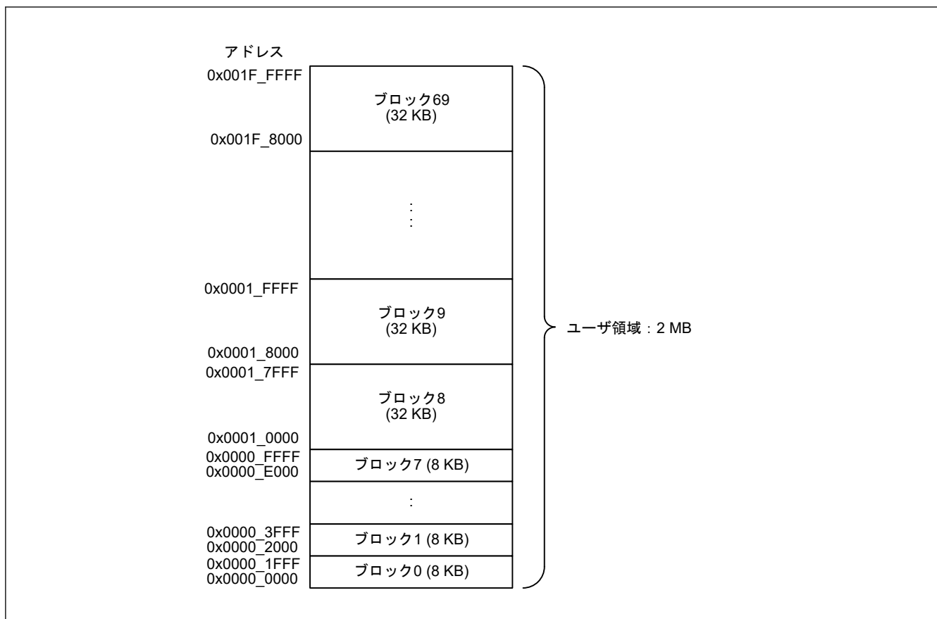
図 50.2 コードフラッシュメモリのマップ
