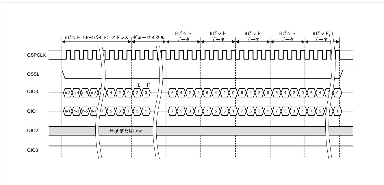
図 35.24 XIP モード時のファストリード Dual I/O バスサイクル
