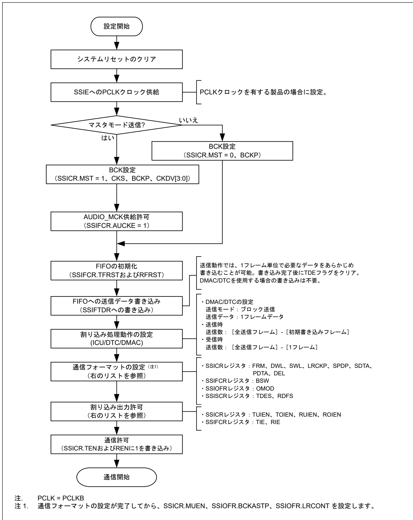
図 38.53 通信開始手順 (CPU 動作手順)
