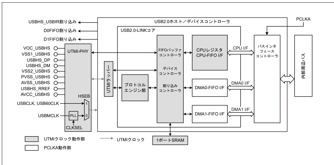
図 29.1 USBHS ブロック図
