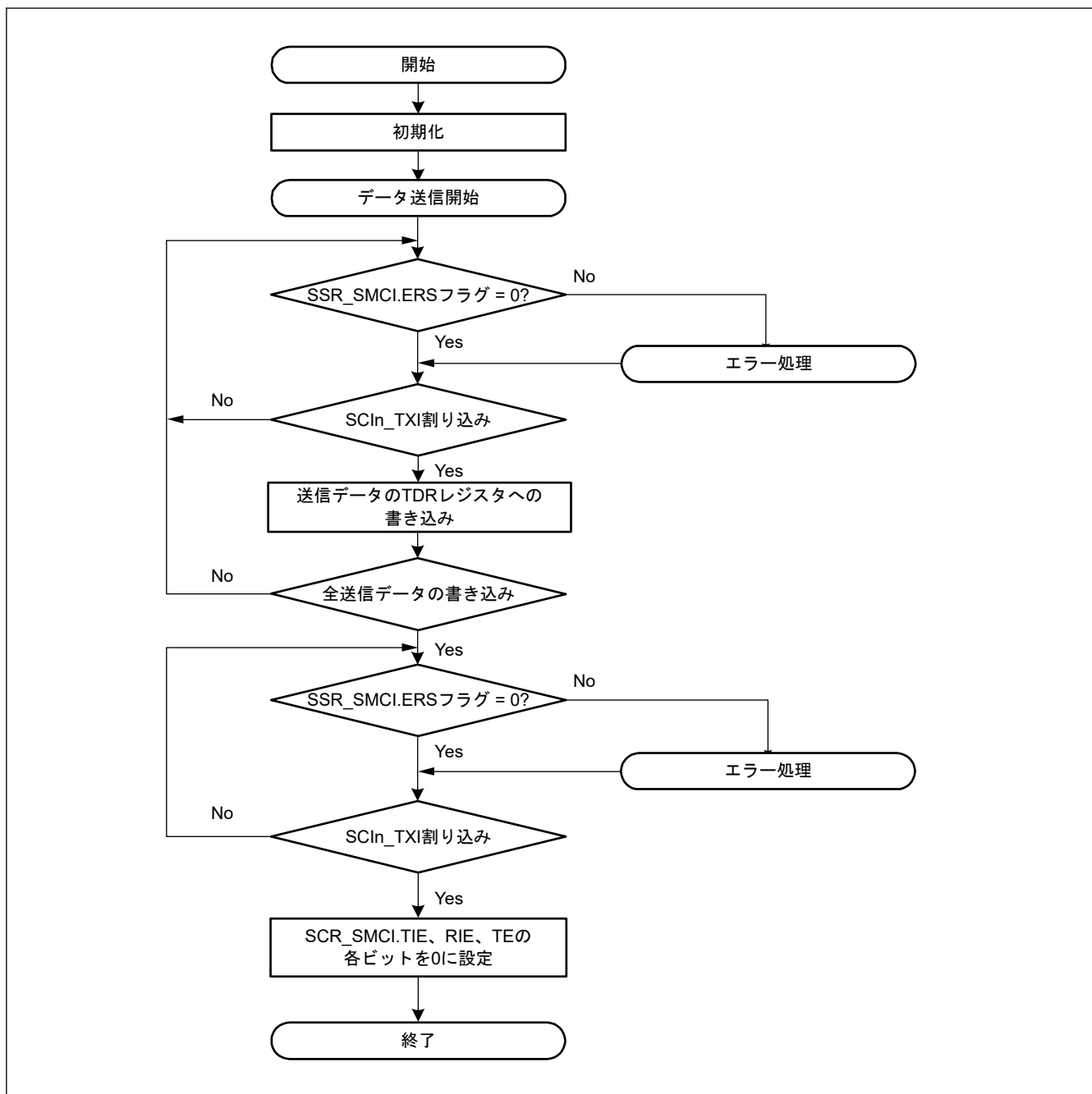
図 30.84 スマートカードインタフェース送信のフローチャート例
