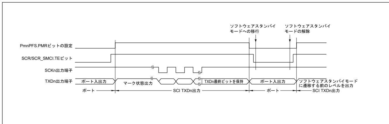
図 30.120 ソフトウェアスタンバイモード遷移中のポートの端子状態 (内部クロック、クロック同期式送信)
