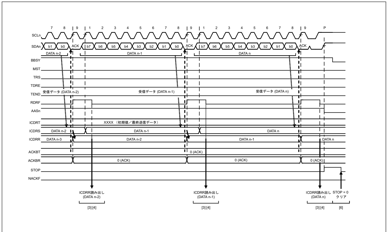
図 31.20 スレープ受信の動作タイミング (2) (RDRFS = 0の場合)
