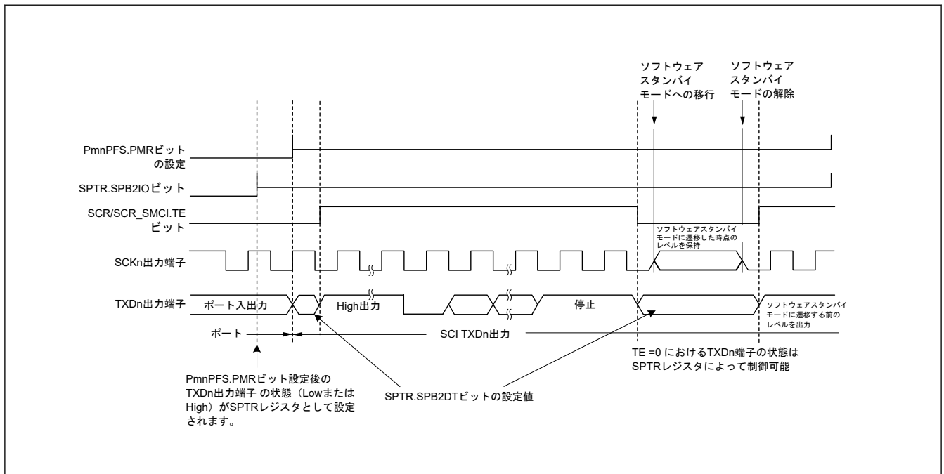
図 30.119 ソフトウェアスタンバイモード遷移中のポートの端子状態 (内部クロック、調歩同期式送信)
