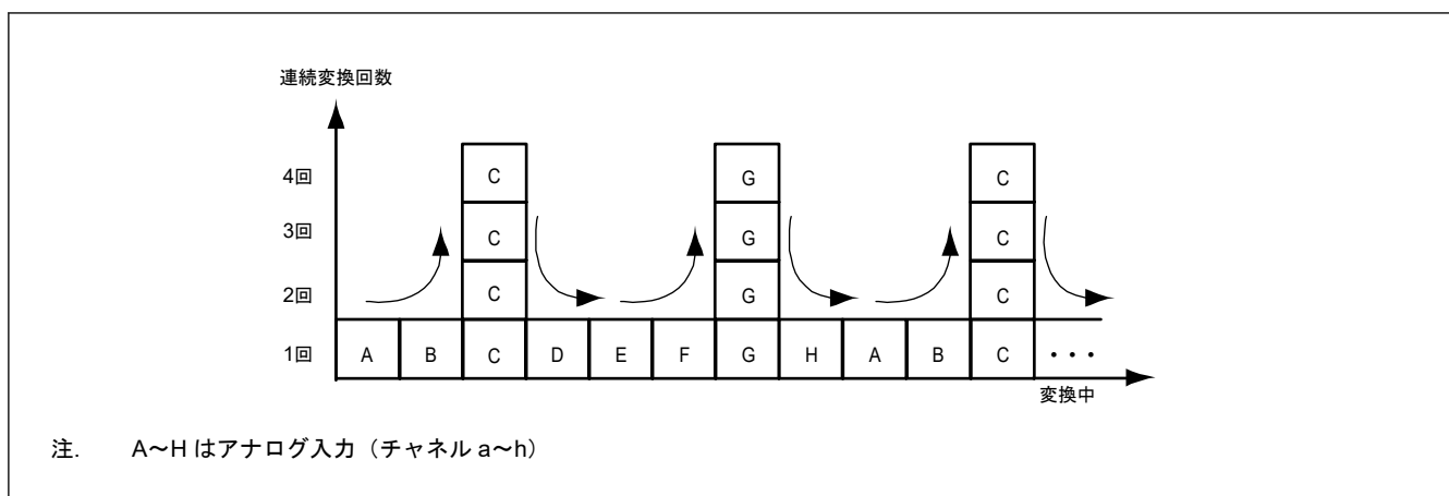
図 43.3 ADADC.ADC[2:0] = 011b および ADADS0/1 によるアナログ入力 C と G を 1 に選択時のスキャン変換シーケンス
