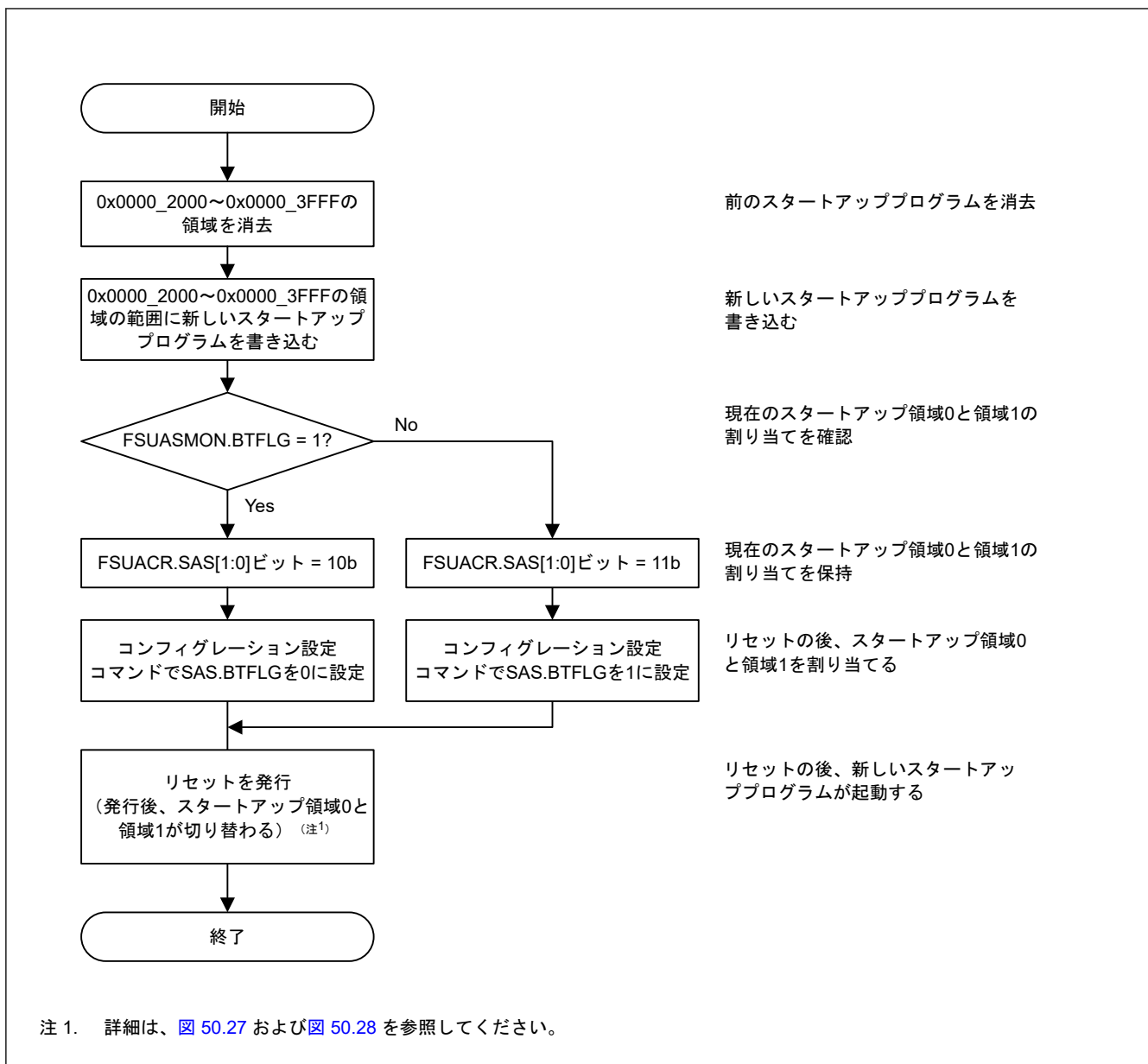
図 50.29 スタートアッププログラムプロテクションの概念
