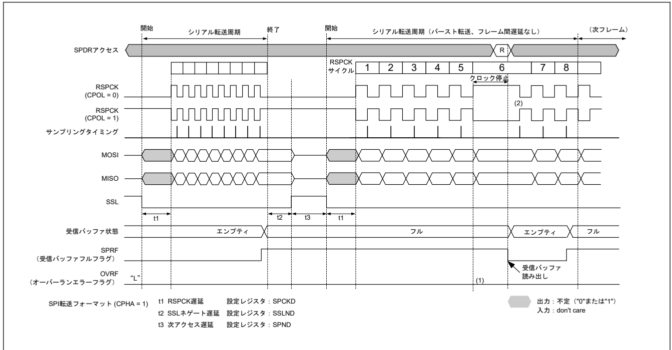
図 34.40 マスタモードの受信バッファフル状態でシリアル転送が継続する場合のクロック停止波形 (バースト転送でフレーム間遅延なし、CPHA = 1)
