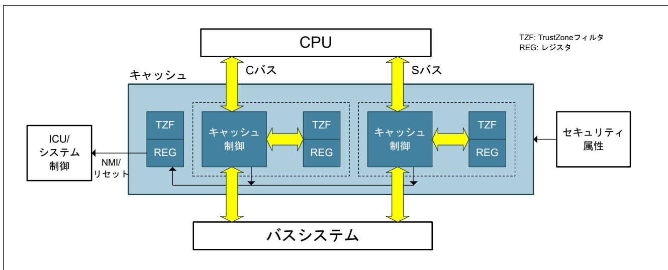
図 14.39 キャッシュのブロック図
