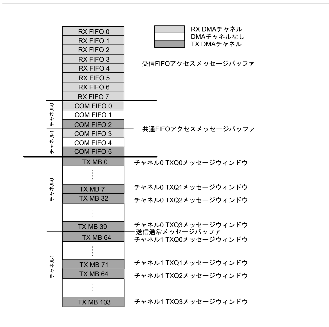
図 32.32 DMA チャンネルに接続可能なメッセージバッファ
