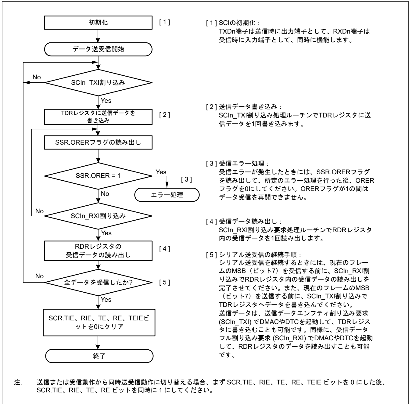
図 30.75 クロック同期式モードにおけるシリアル同時送受信動作のフローチャート例（非 FIFO 選択時）
