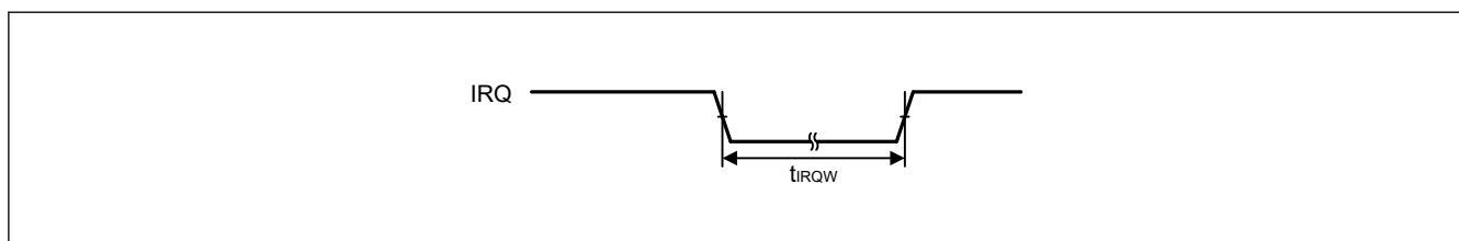
図 53.19 IRQ 割り込み入カタイミング
