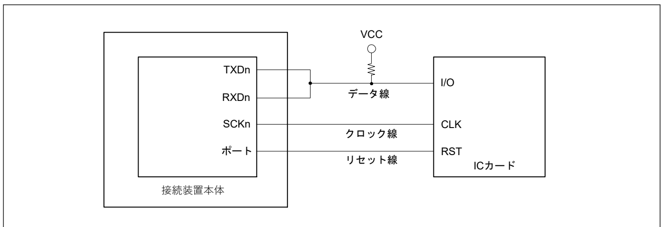
図 30.77 スマートカード (IC カード) との接続例
