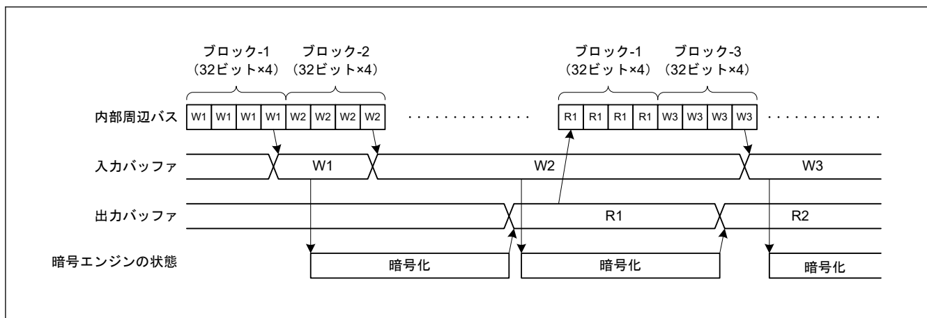
図 42.3 暗号/復号処理タイミング (AES)
