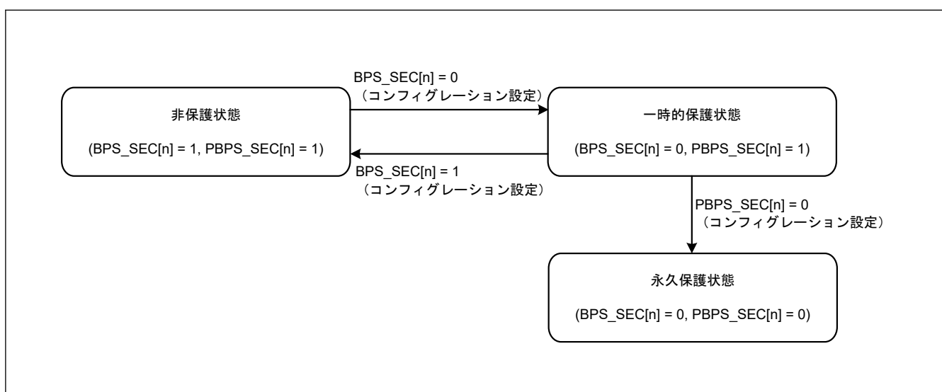
図 50.35 BPS_SEC[n]ビットおよび PBPS_SEC[n]ビットによるフラッシュシーケンサの状態遷移
