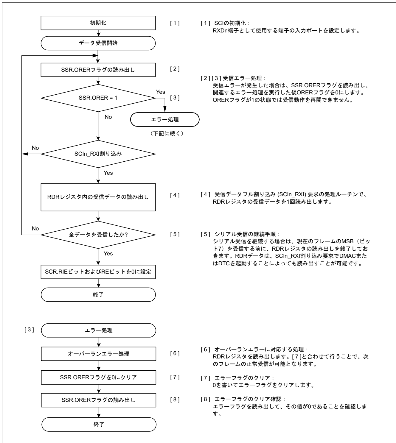
図 30.73 クロック同期式モードにおけるシリアル受信のフローチャート例 (非 FIFO 選択時)
