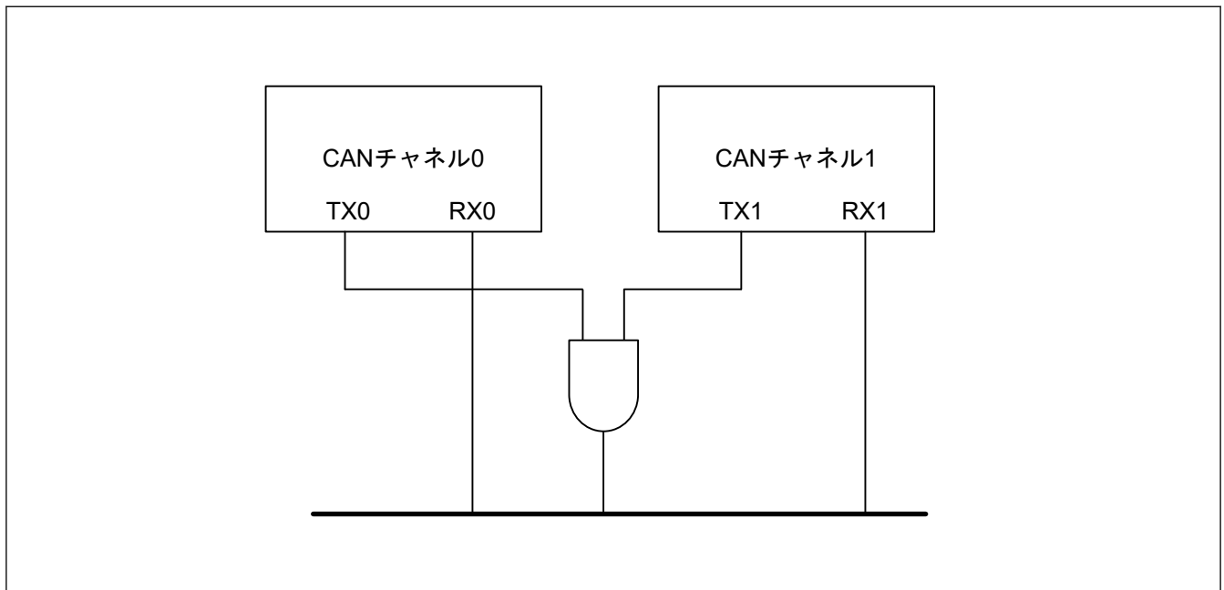
図 32.53 内部 CAN バスの接続
