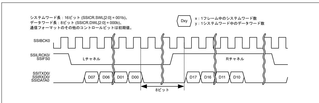
図 38.36 パディングビット転送の例 (I 2 S フォーマット、システムワード長 > データワード長)
