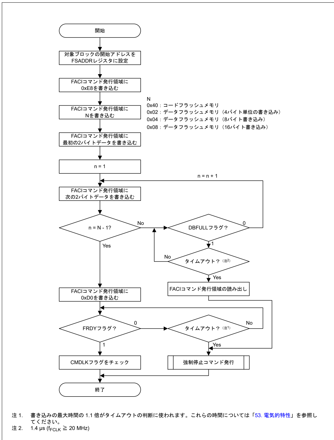
図 50.14 プログラムコマンドの使用フロー
