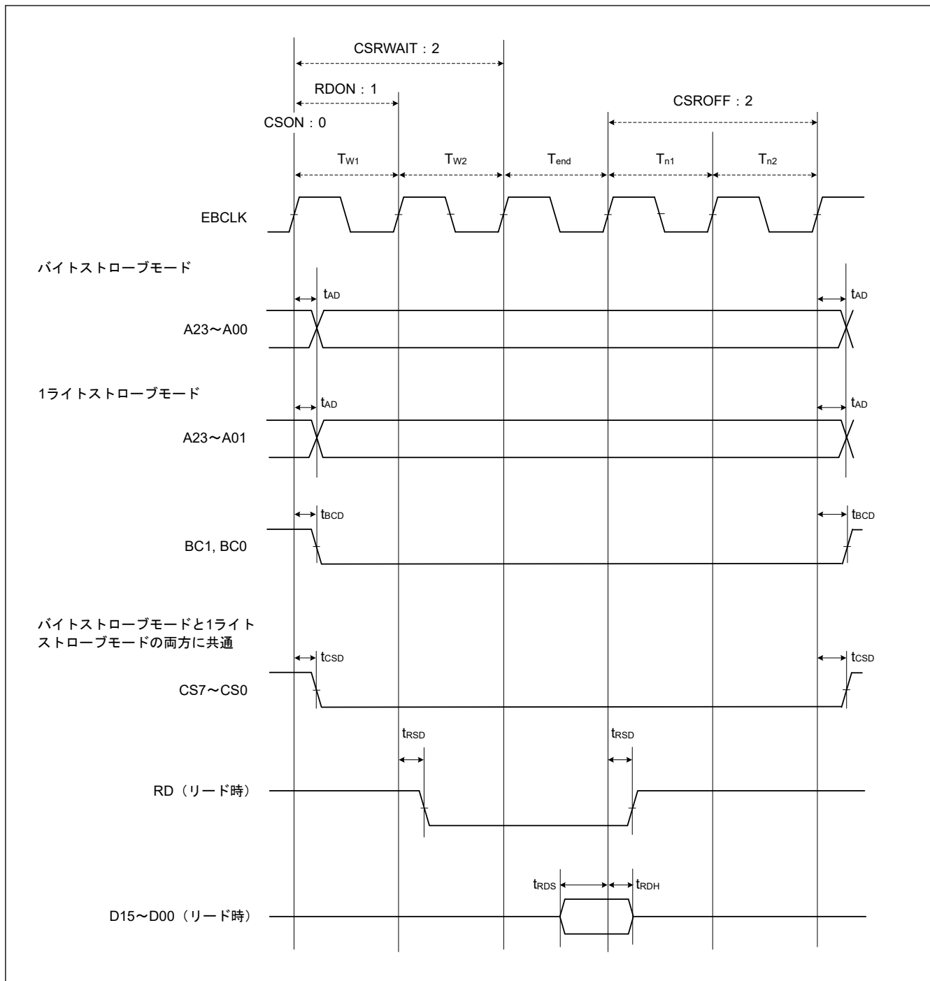
図 53.22 バスクロック同期を使用したノーマルリードサイクルの外部バスタイミング
