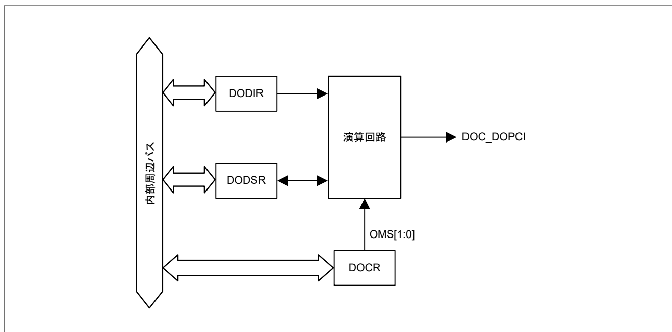
図 47.1 DOC のブロック図
