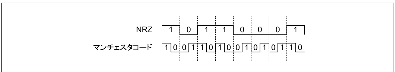
図 30.49 マンチェスタエンコードの例
