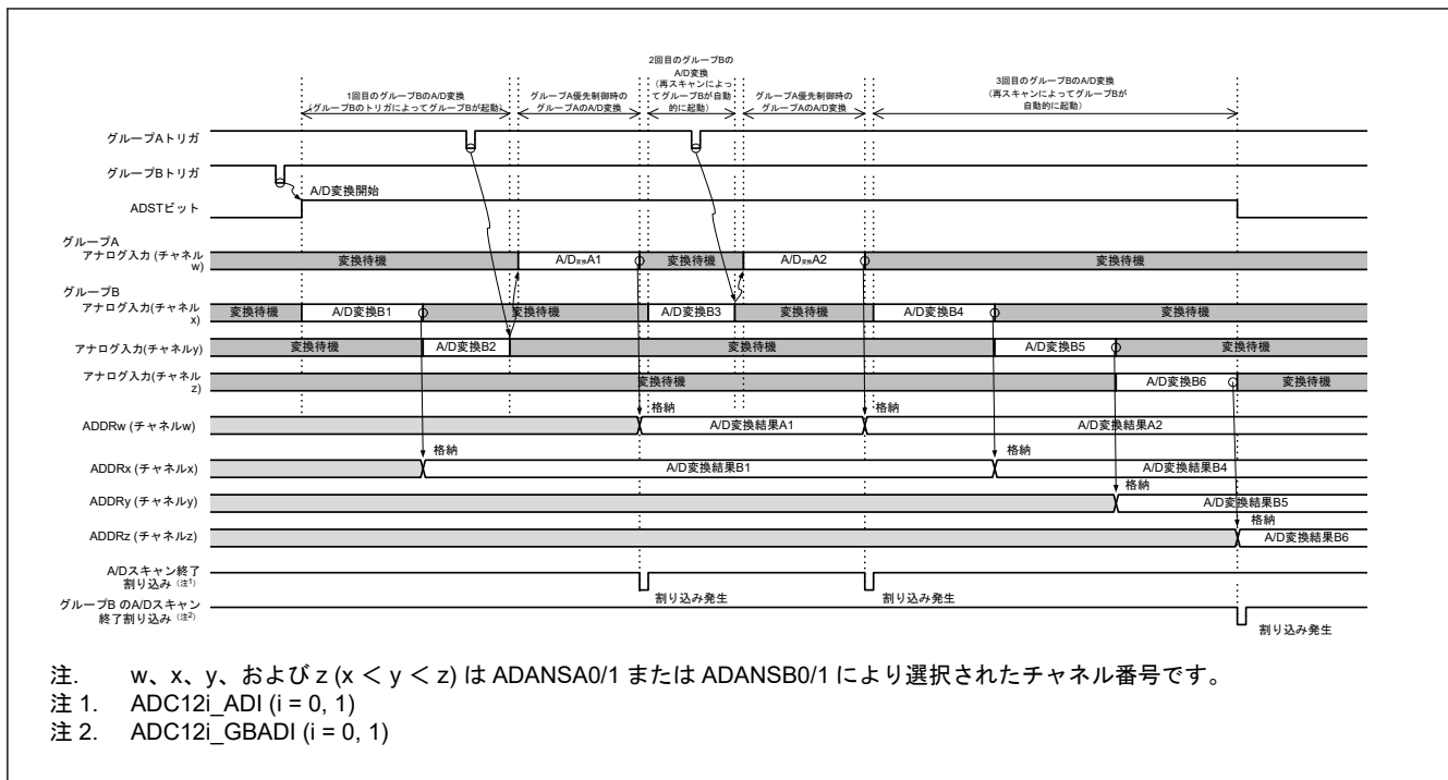
図 43.20 グループ優先動作の例 1-2 : グループ B 再スキャン中のグループ A トリガ入力、再スキャンあり (ADGSPCR.GBRSCN = 1、ADGSPCR.GBRP = 0、および ADGSPCR.LGRRS = 0 の場合)
