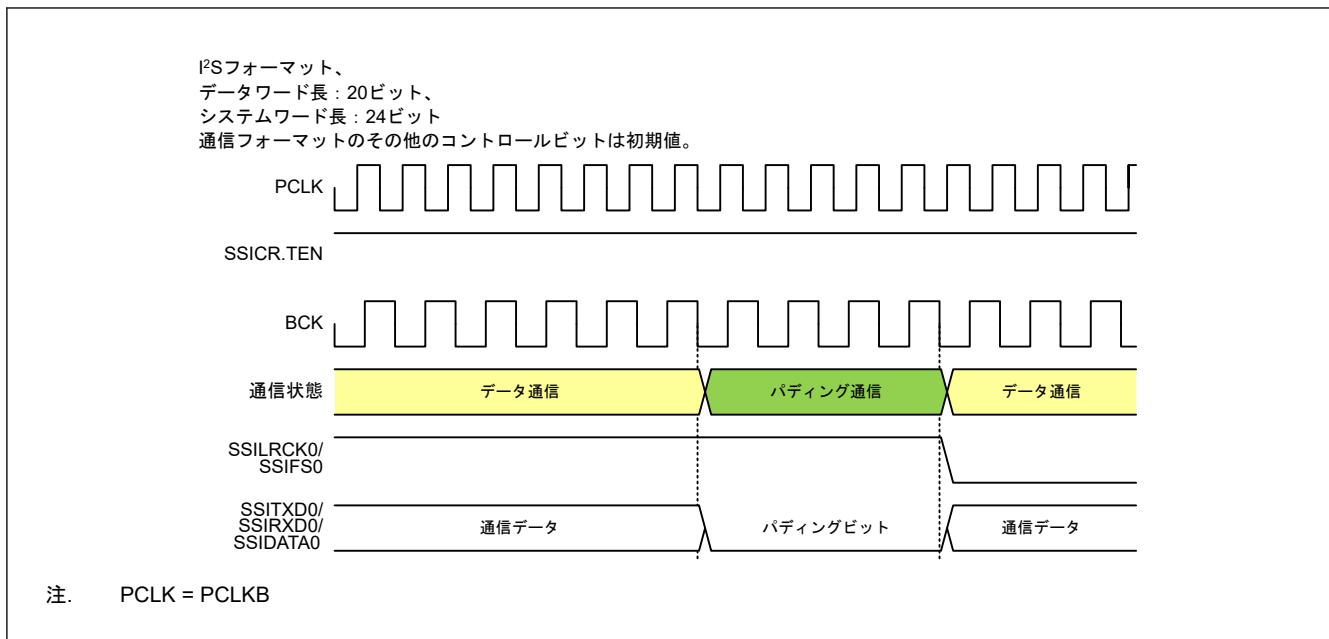
図 38.49 データ通信からパディング通信への遷移
