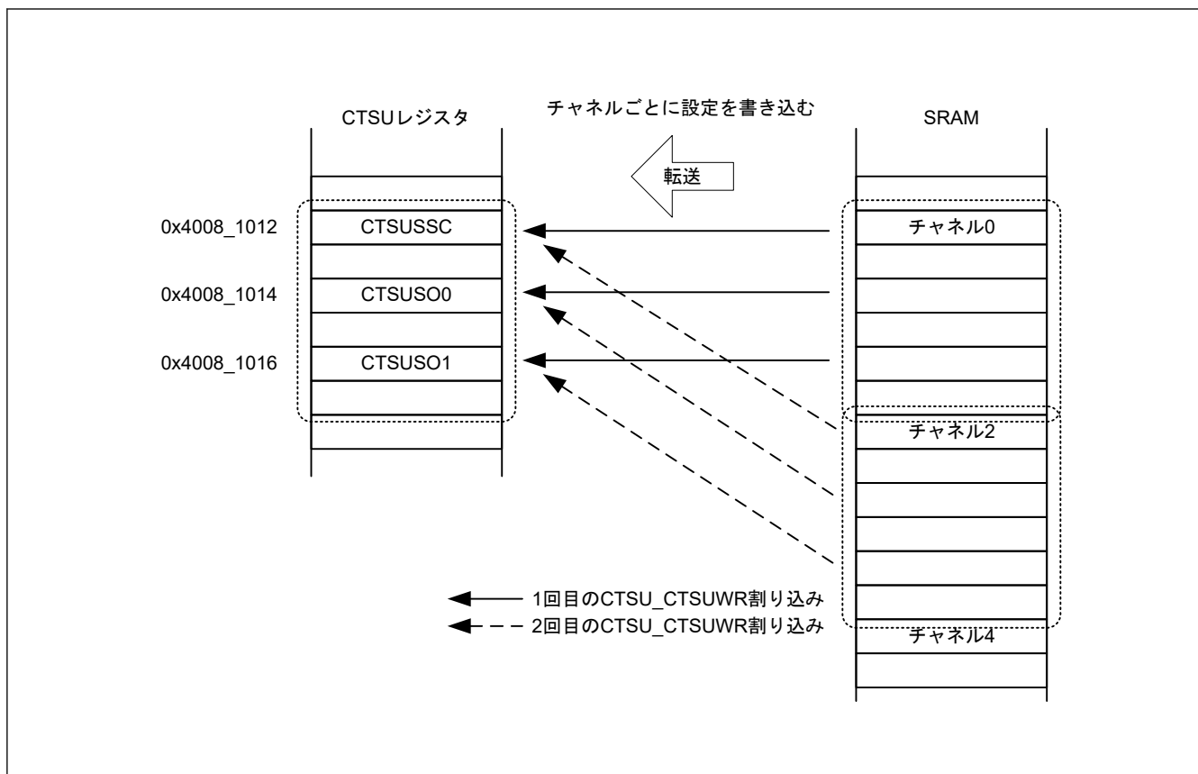
図 46.19 CTSU_CTSUWR 割り込みを用いた DTC 転送動作例
