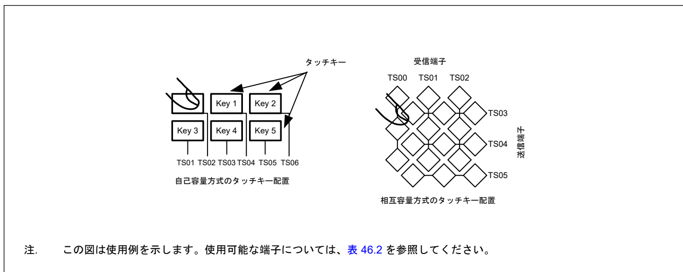
図 46.8 自己容量方式と相互容量方式の概要
