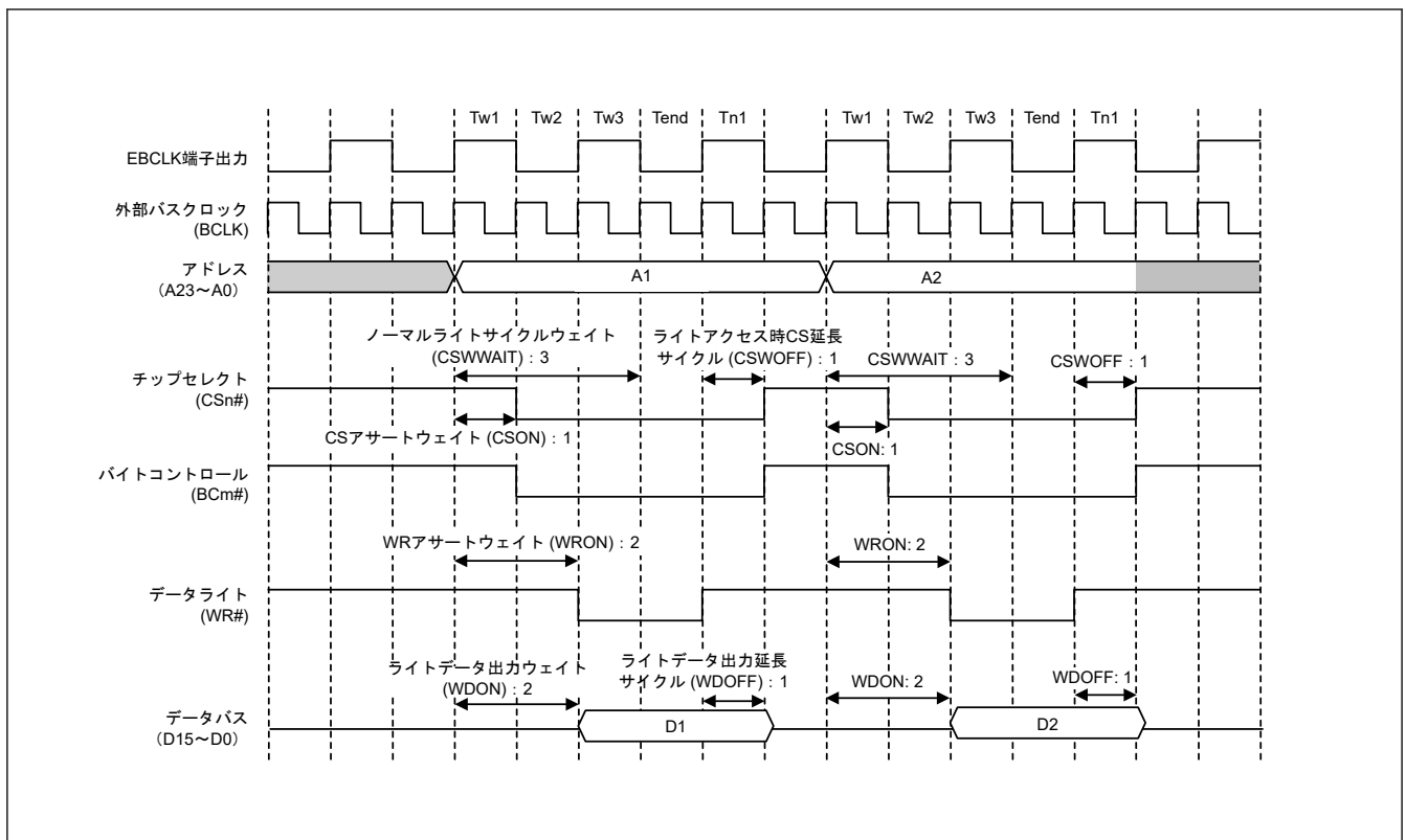
図 14.14 ノーマルライトアクセスの動作例 (EBCLK 端子出力選択ビットで BCLK の 2 分周を設定した場合) (n = 0~7、m = 0~1)
