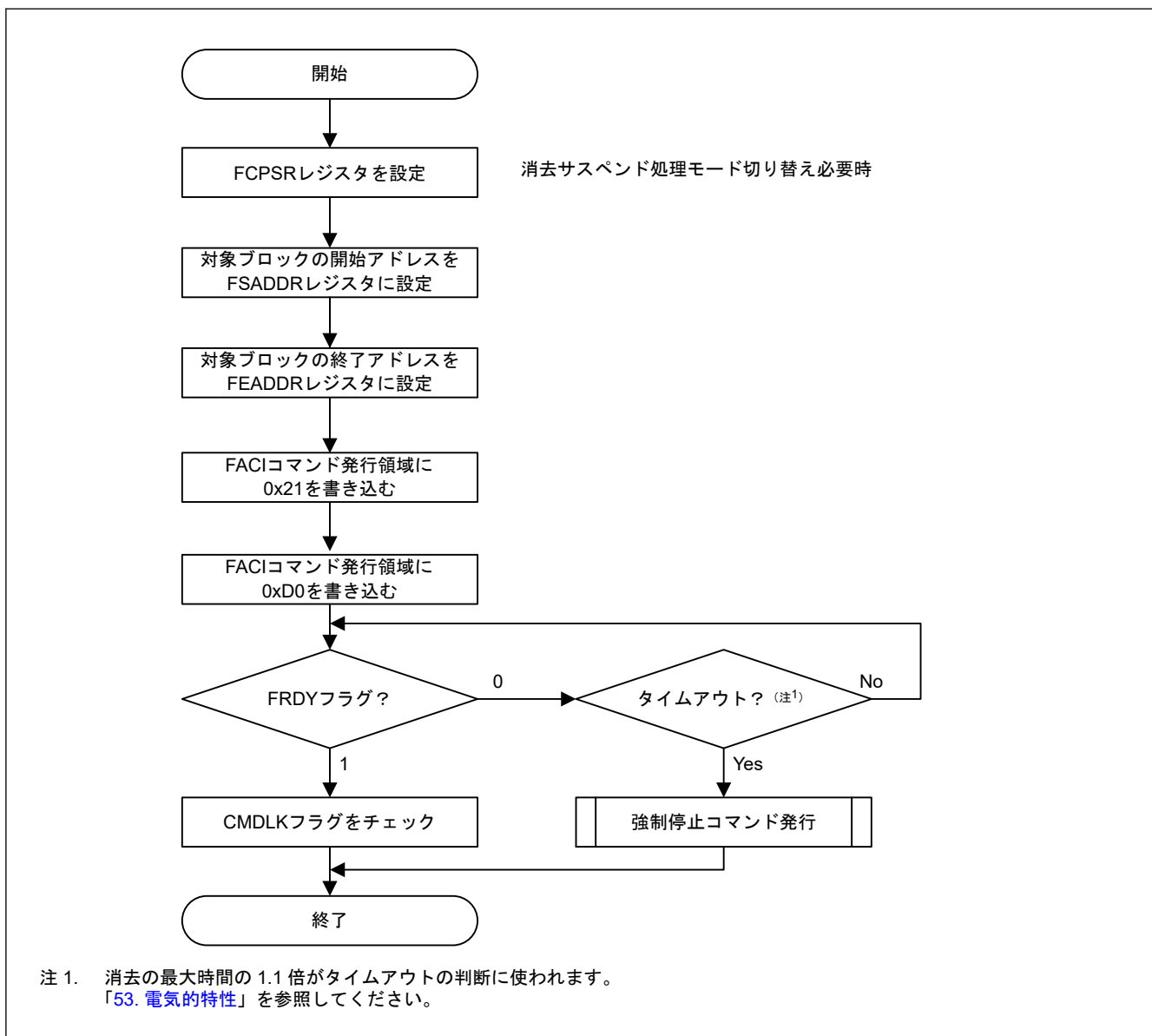
図 50.16 マルチブロックコマンドの使用フロー
