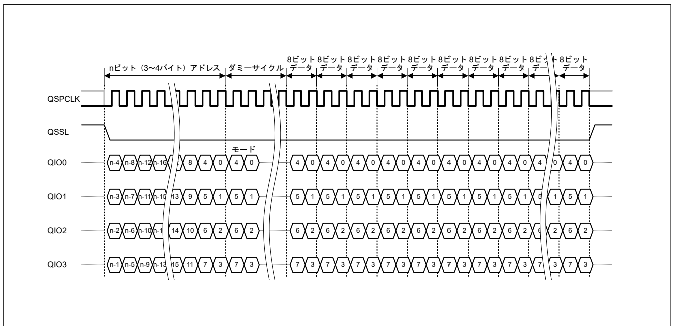
図 35.28 XIP モード時のファストリード Quad I/O パスサイクル
