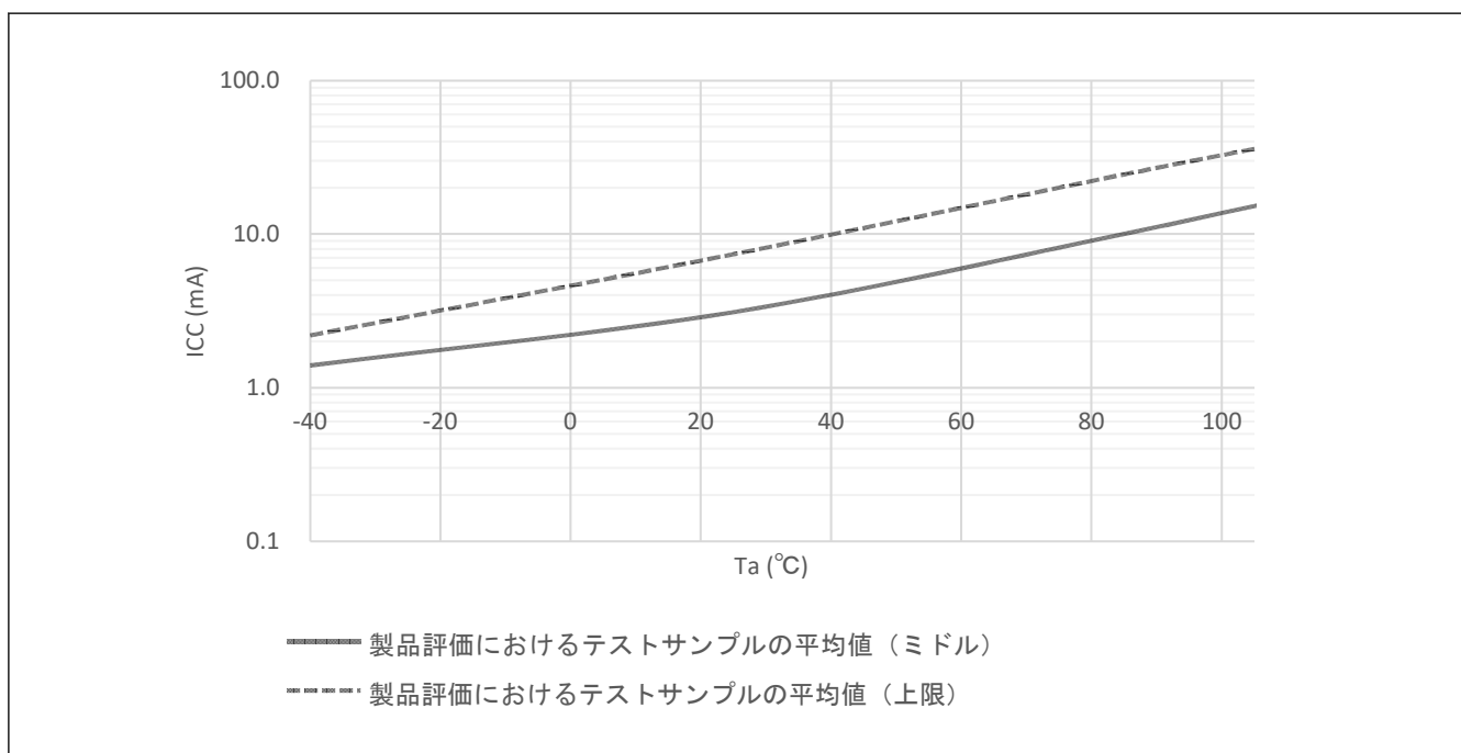
図 53.2 ソフトウェアスタンバイモード時の温度依存性 (参考データ)
