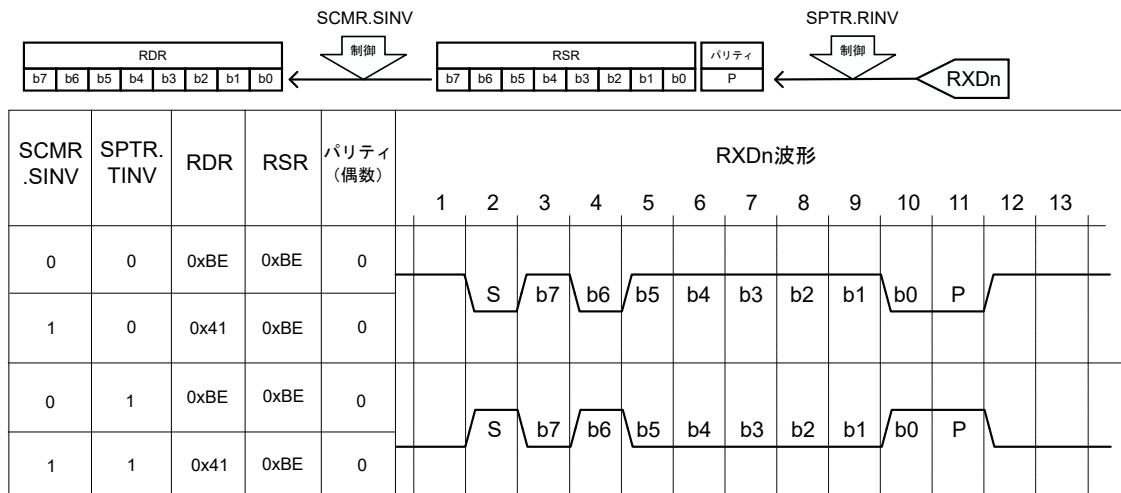
図 30.5 受信/送信データ制御の例
