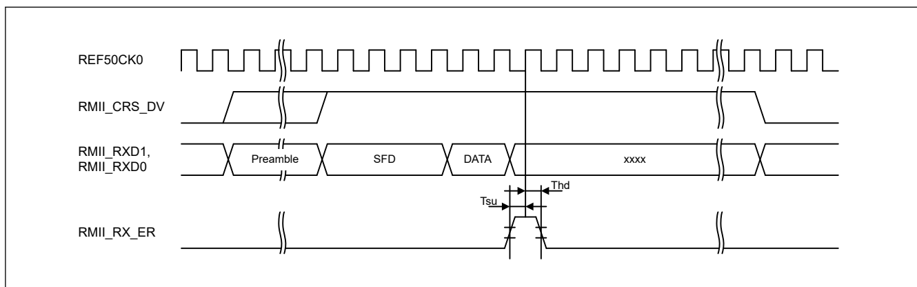
図 53.67 エラー発生時の RMIi 受信タイミング
