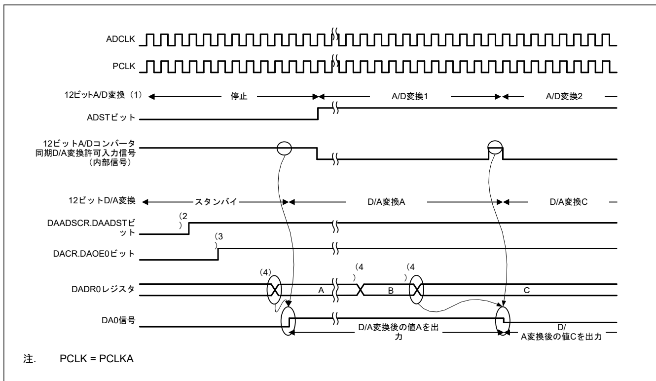
図 44.3 DAC12 を次に同期して変換する例：ADC12 (ユニット 1)
