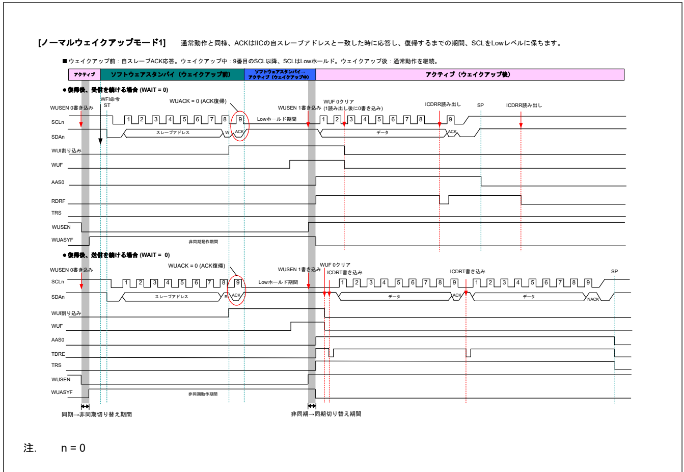
図 31.32 ノーマルウェイクアップモード1のタイミング
