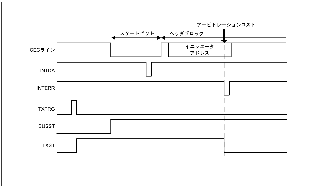
図 37.27 アービトレーションロスト発生時の送信ステータスフラグのタイミング
