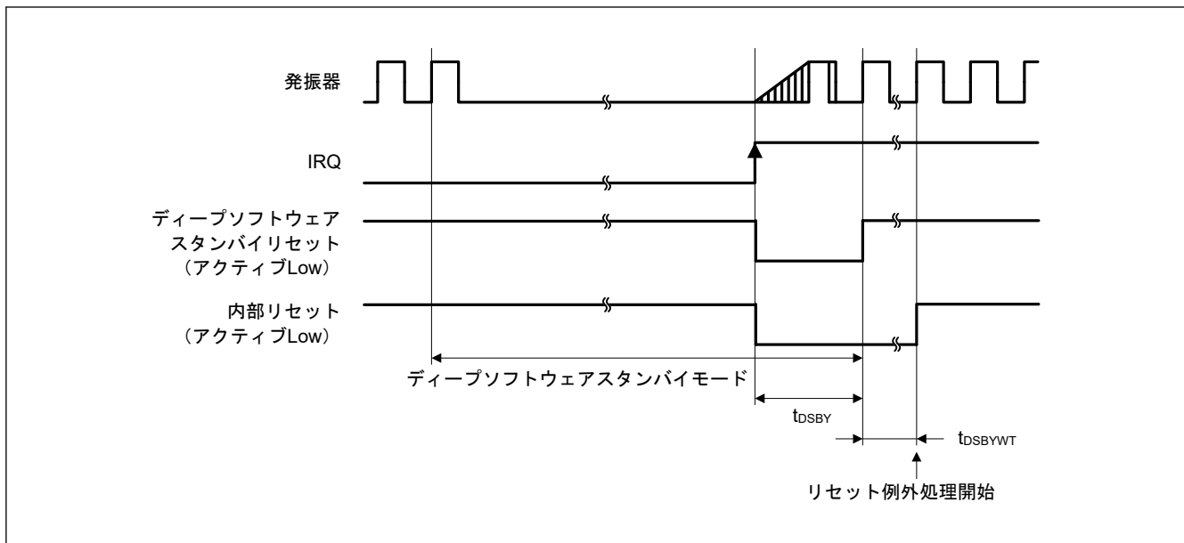
図 53.16 ディープソフトウェアスタンバイモード解除タイミング
