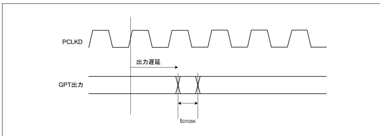
図 53.31 OPS の GPT 出力遅延スキュー
