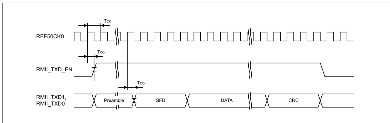
図 53.65 RMIi 送信タイミング
