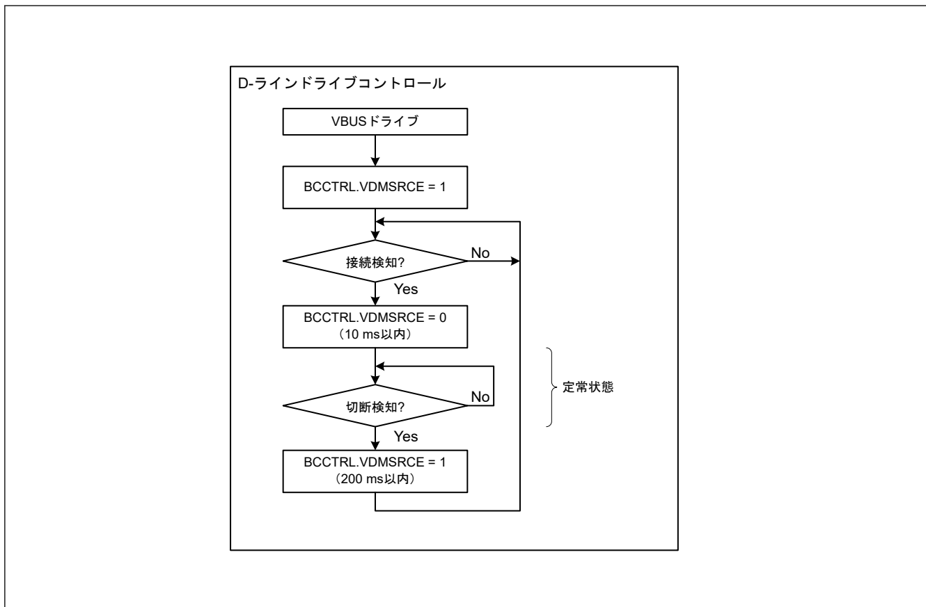
図 29.20 ハードウェアに Portable Device 検出機能未搭載または未使用時の Charging Downstream ポート処理フロー
