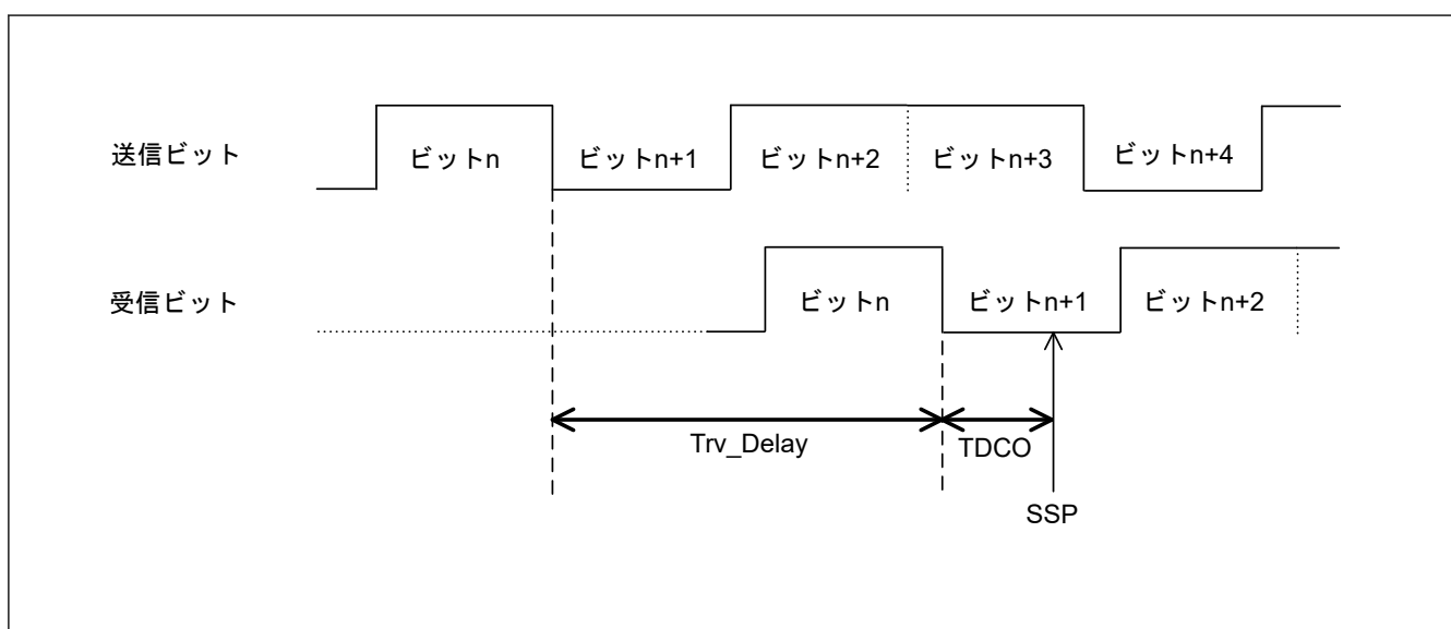
図 32.20 セカンダリサンプルポイントの位置
