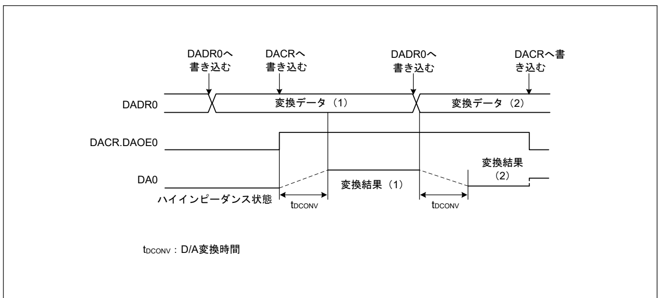
図 44.2 DAC12 の動作例
