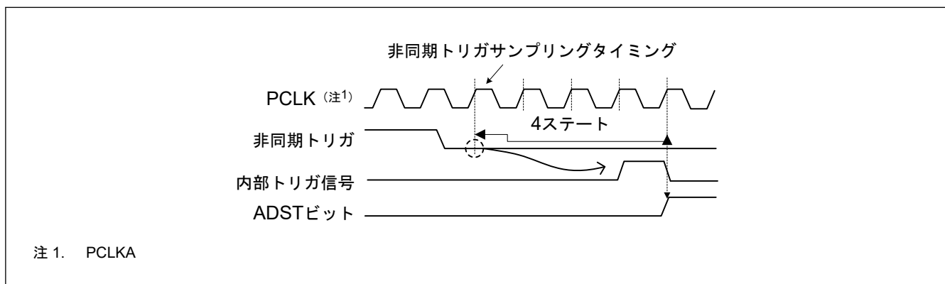
図 43.36 非同期トリガ入力タイミング
