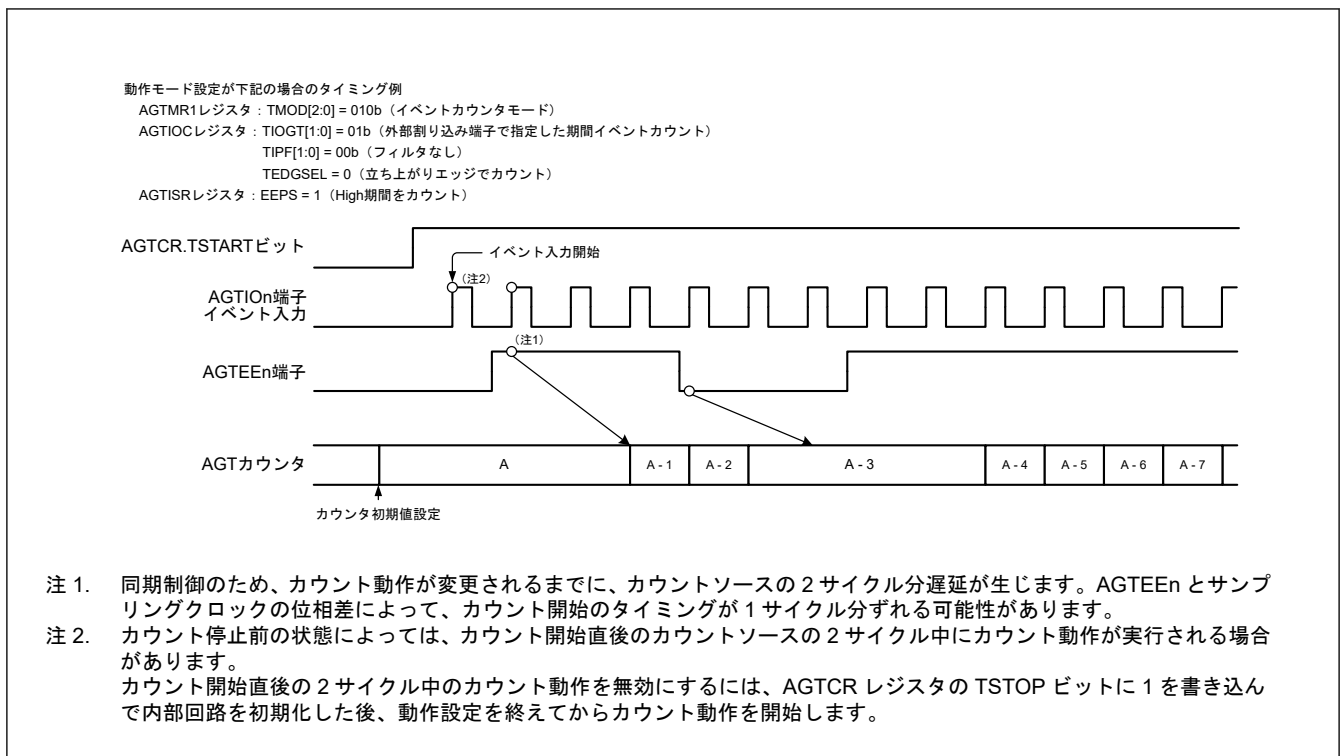
図 22.9 イベントカウントモードでの動作例 2
