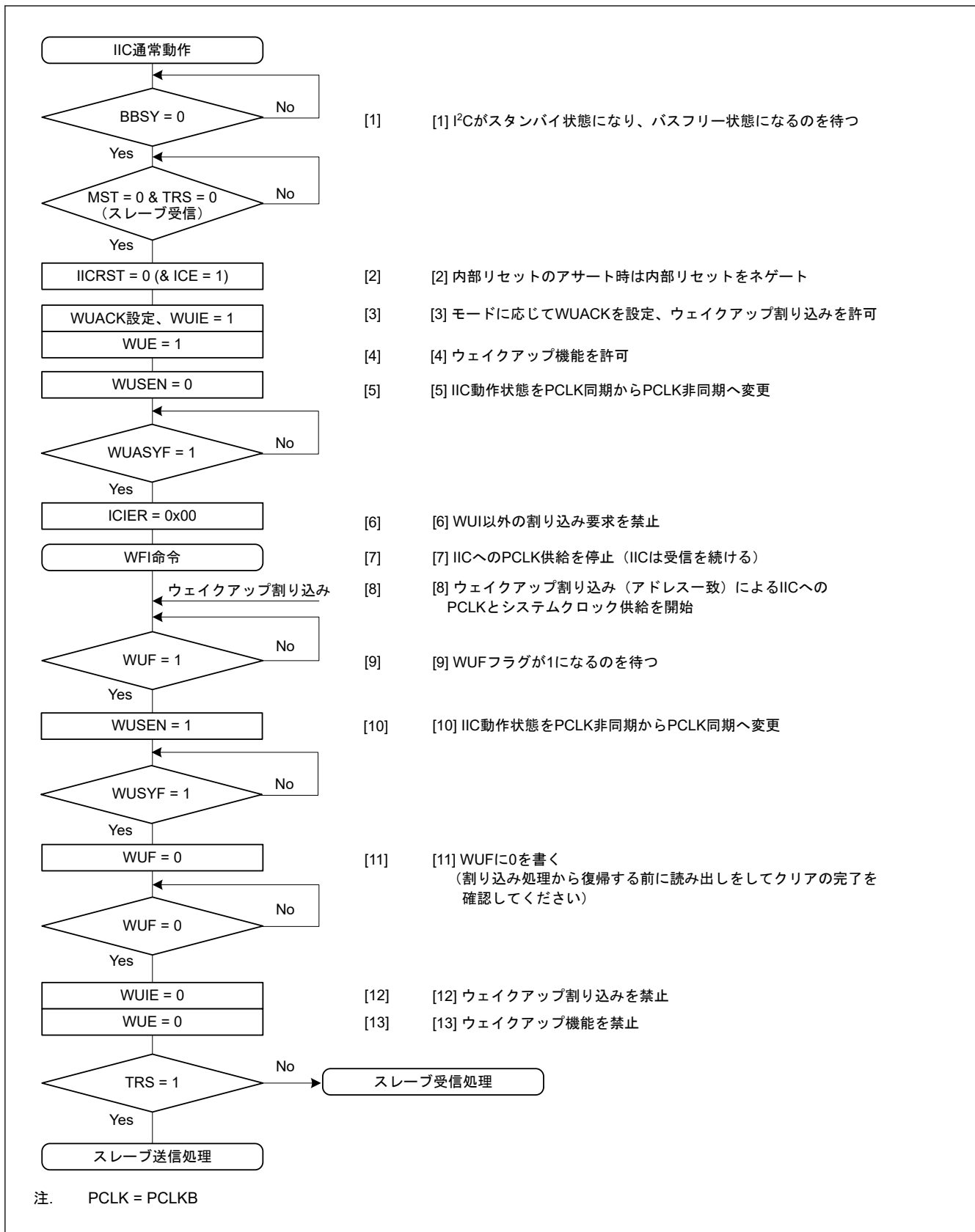
図 31.33 ノーマルウェイクアップモード2の動作例 (スレーブアドレス一致時のウェイクアップ割り込みによるウェイクアップの場合)
