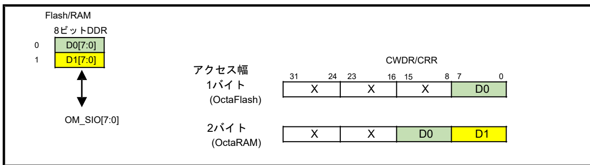
図 36.12 OctaFlash および OctaRAM スペースの構成レジスタデータアラインメント
