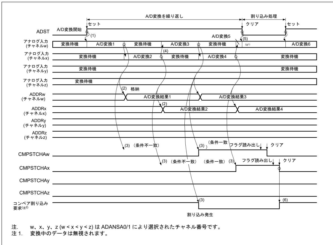
図 43.28 コンペア機能の動作例 (アナログ入力 (チャンネル w~z) を比較)
