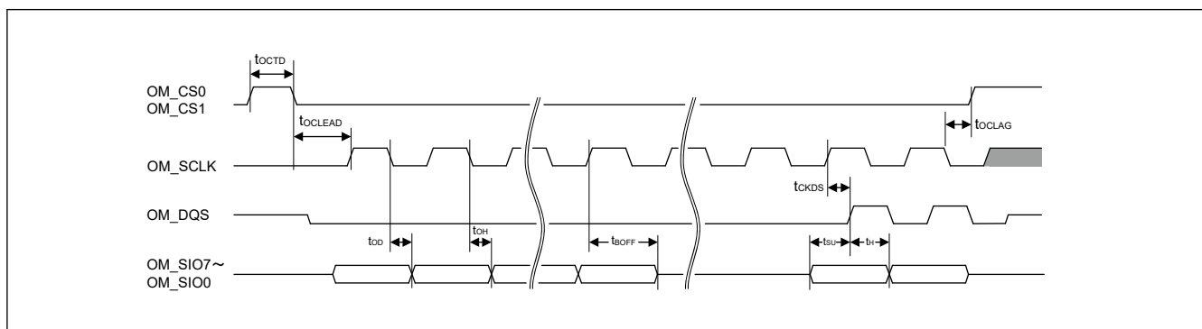
図 53.53 SOPI 転送フォーマット送受信タイミング
