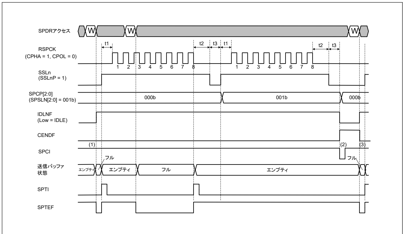
図 34.31 通信終了割り込み動作例（送受信／送信マスターモード）
