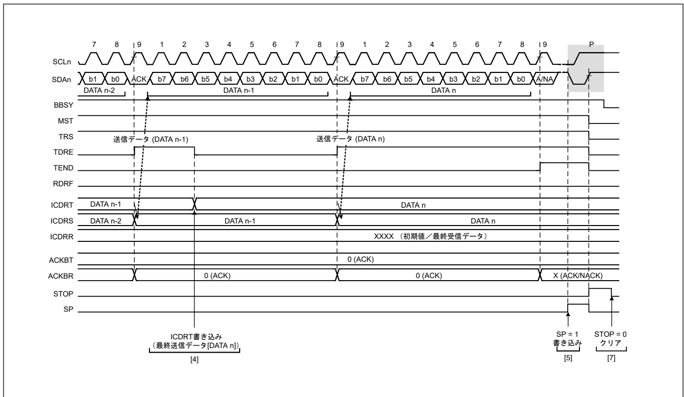
図 31.9 マスタ送信の動作タイミング (3)
