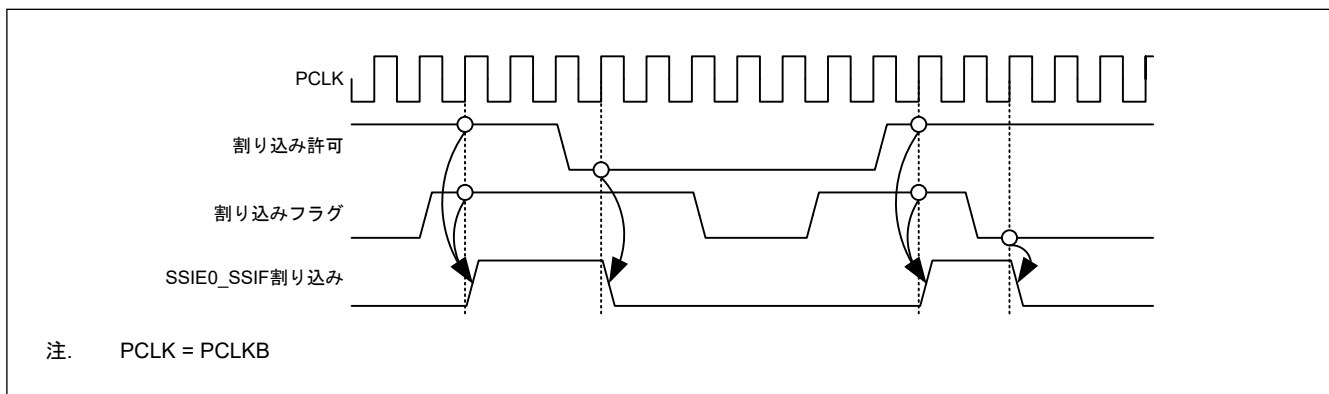
図 38.59 共通割り込み要因のタイミング図 (SSIE0_SSIF)
