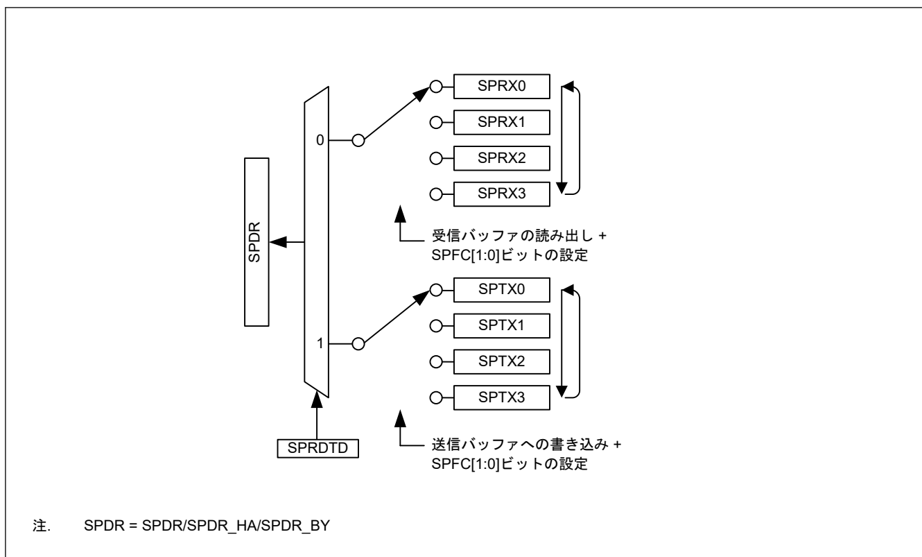
図 34.4 読み出し時の SPDR/SPDR_HA/SPDR_BY レジスタの構成図
