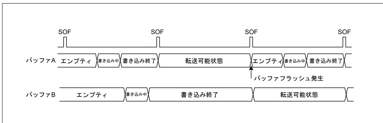
図 29.17 バッファフラッシュ動作例
