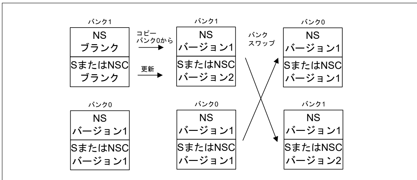
図 52.4 セキュア領域または NSC 領域のフィールドアップデートフロー
