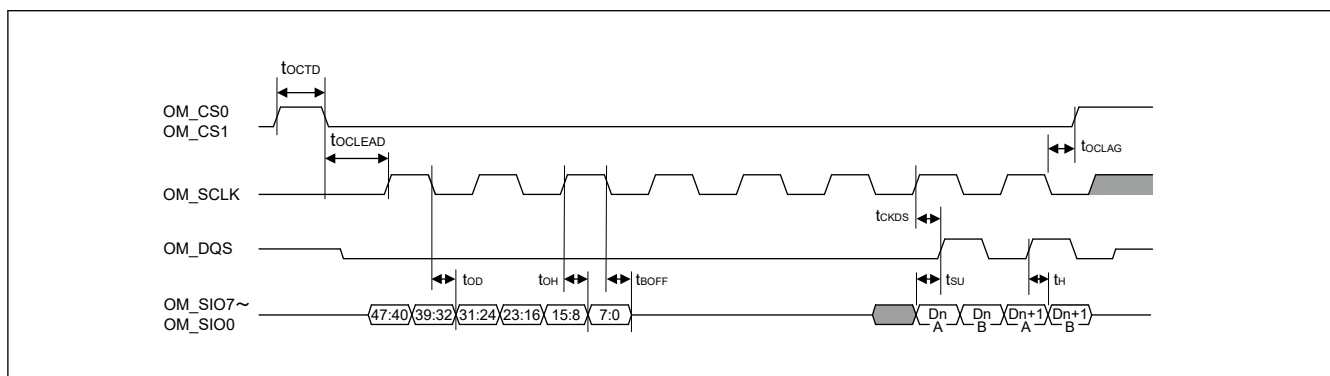
図 53.54 DOPI 転送フォーマット送受信タイミング
