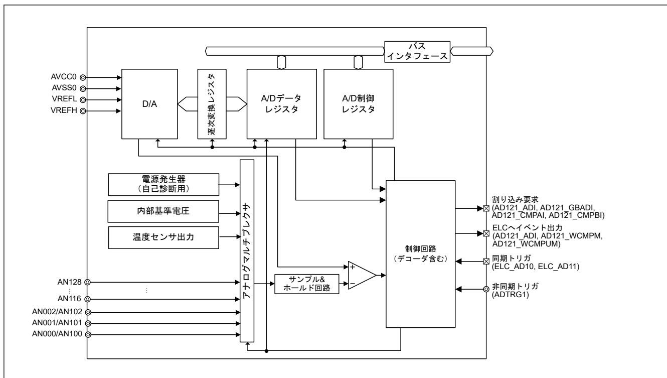
図 43.2 ADC12 のブロック図 (ユニット 1)
