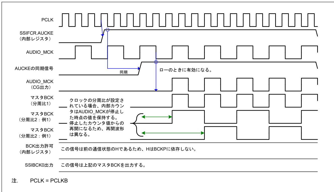
図 38.27 通信停止からマスタモード通信開始までの動作のタイミング図
