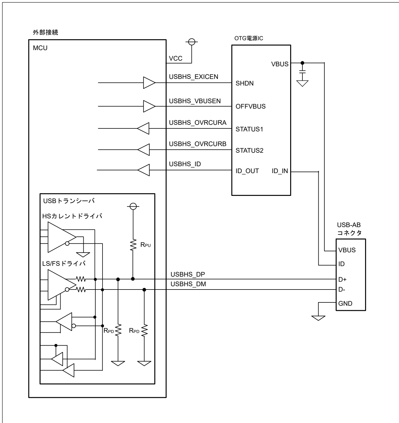
図 29.27 セルフパワーシステムでの OTG 接続例
