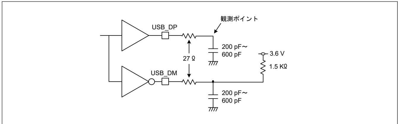
図 53.75 Low-speed モードにおける測定回路
