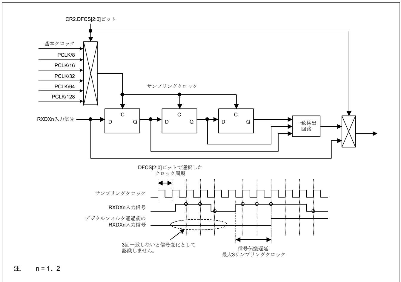
図 30.112 デジタルフィルタ機能の動作例
