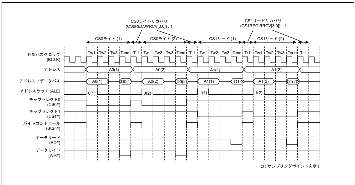
図 14.32 バスアクセスが分割された場合のリカバリサイクルの動作例 (セパレートバスインタフェース、ノーマルアクセスの場合) (m = 0~1)
