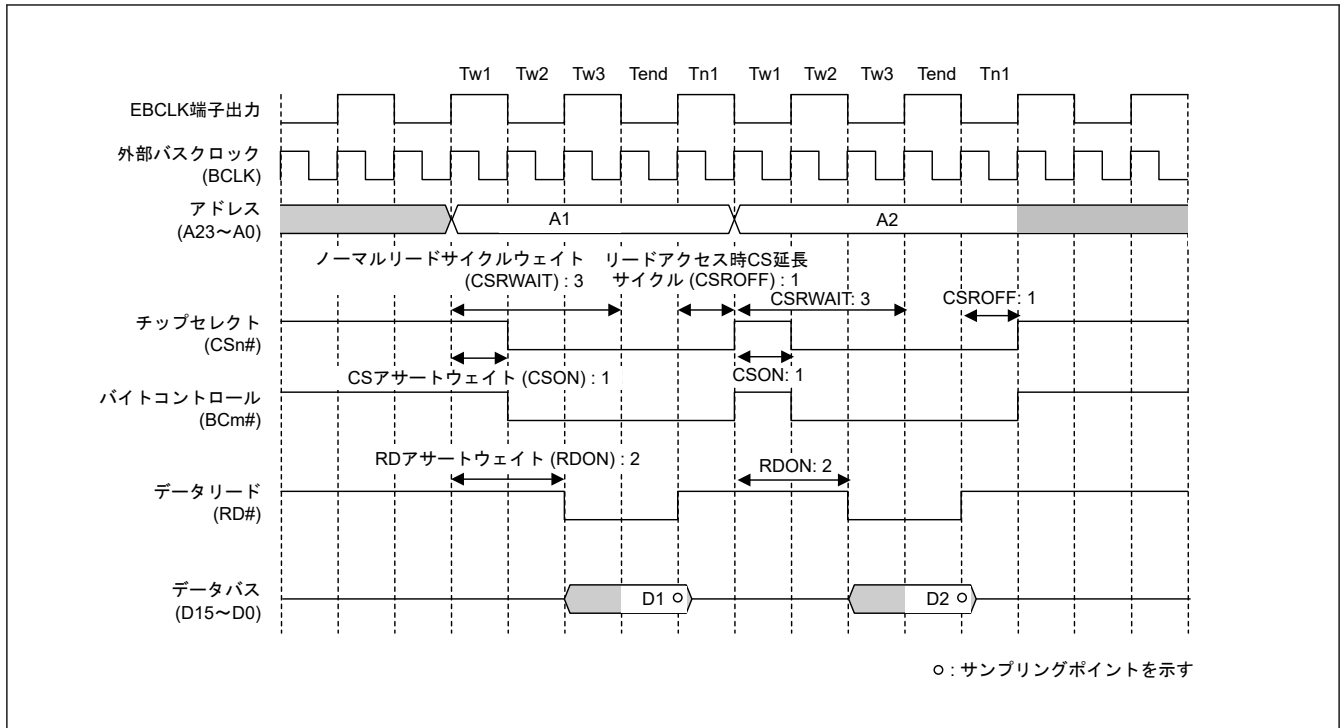
図 14.15 ノーマルリードアクセスの動作例 (EBCLK 端子出力選択ビットで BCLK の 2 分周を設定した場合、および 1 転送要求に対して 2 回バスアクセスが発生する場合) (n = 0~7、m = 0~1)
