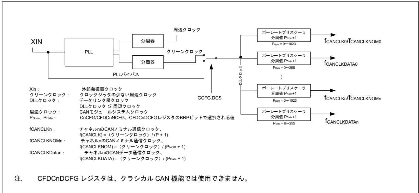
図 32.16 CAN チャンルの通信クロックを生成する回路のブロック図
