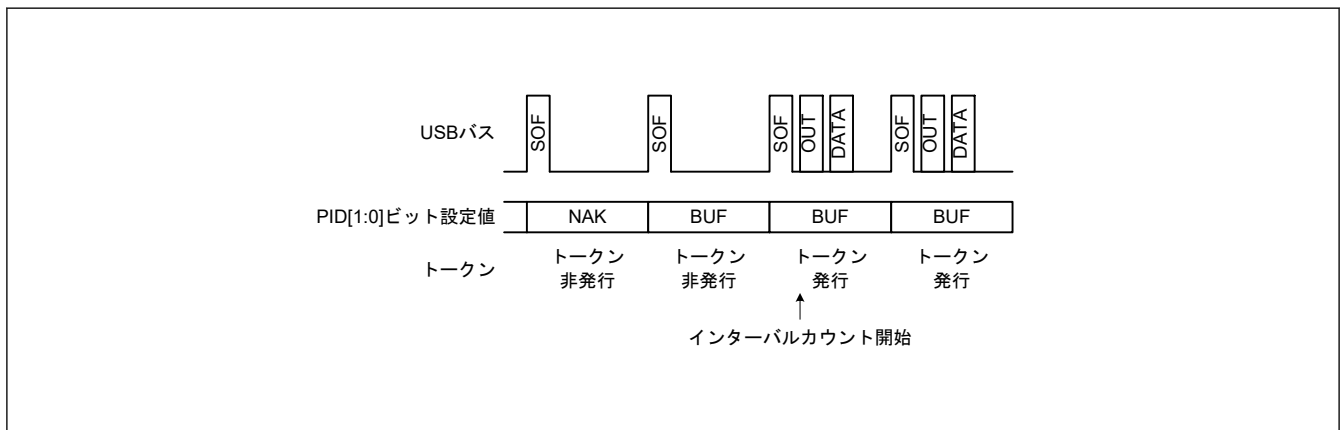
図 29.12 IITV[2:0] = 0 の場合におけるトークン発行の有無
