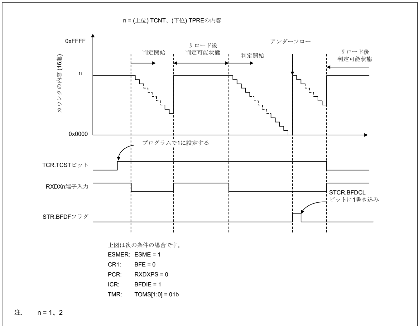
図 30.116 Break Field Low width 判定モードの動作例
