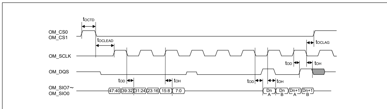
図 53.55 DOPI 転送フォーマット送信タイミング
