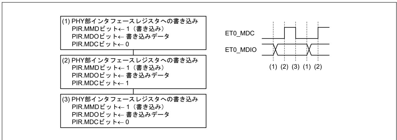
図 26.18 バス解放フロー (表 26.3 の書き込み動作時の IDLE)
