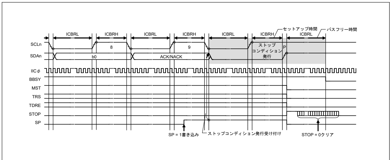
図 31.47 ストップコンディション発行タイミング (SP ビットの使用)
