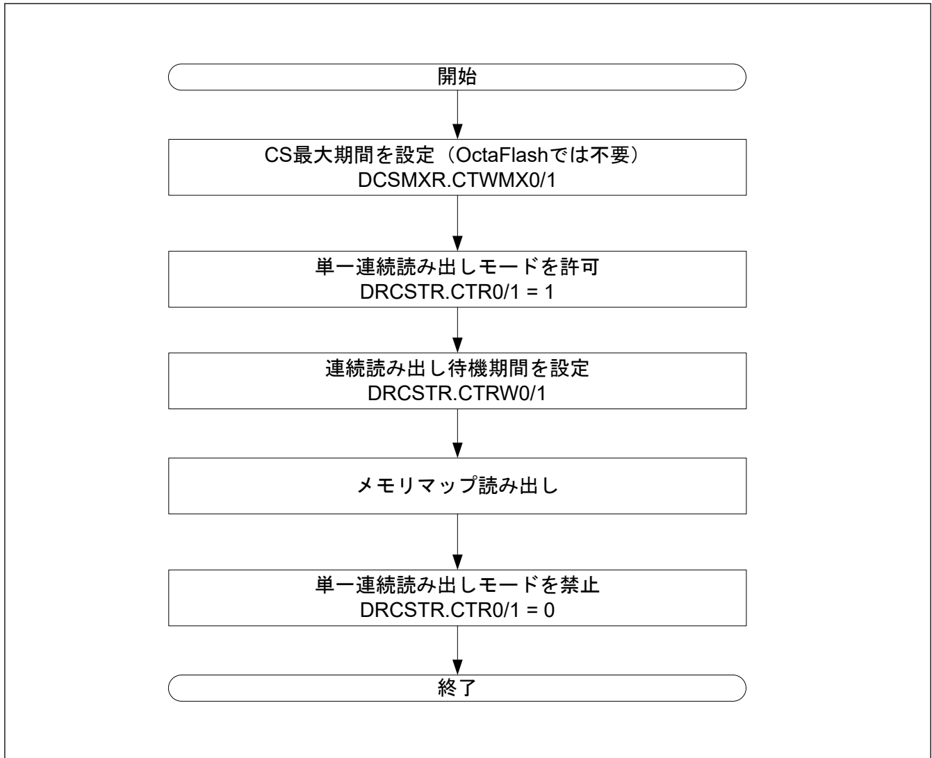
図 36.21 単一連続読み出しの手順
