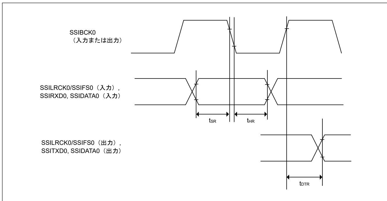
図 53.61 SSICR.BCKP = 1 の場合の SSIE データ送受信タイミング
