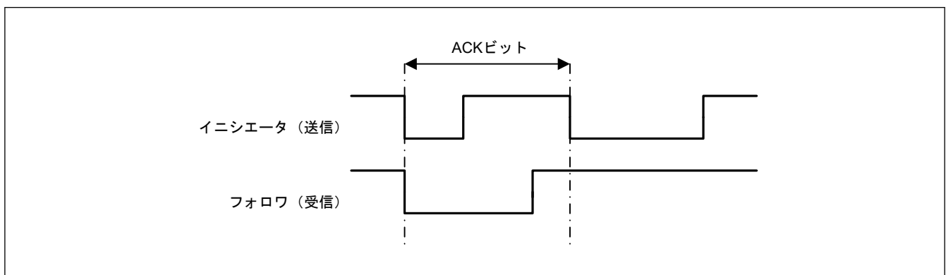
図 37.3 イニシエータ/フォロワー ACK ビット出力例
