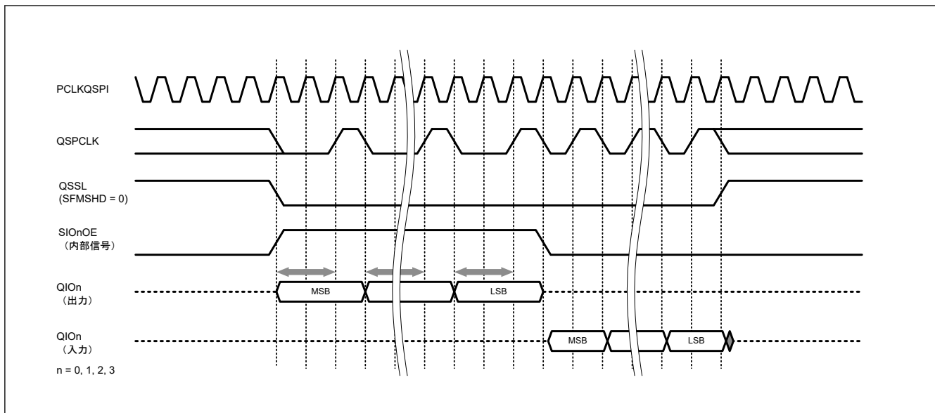
図 35.15 SFMOSW ビットを使用したシリアルデータ出力のセットアップ時間調整
