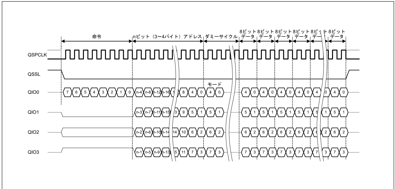
図 35.5 拡張 SPI プロトコル例 (ファストリード Quad I/O)
