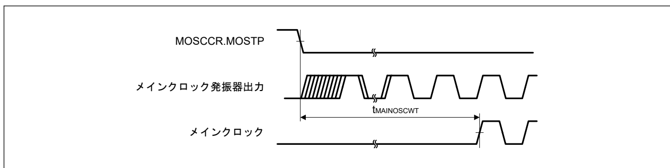
図 53.9 メインクロック発振開始タイミング
