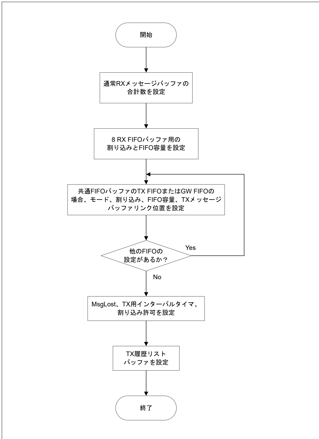
図 32.29 CANFD モジュールにおける FIFO バッファの構成フロー
