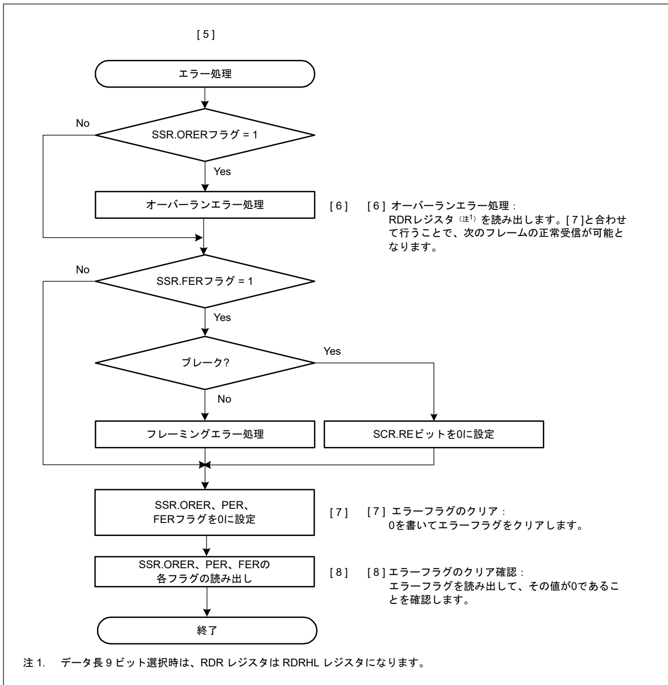
図 30.46 マルチプロセッサシリアル受信のフローチャート例（非 FIFO 選択時）(2)
