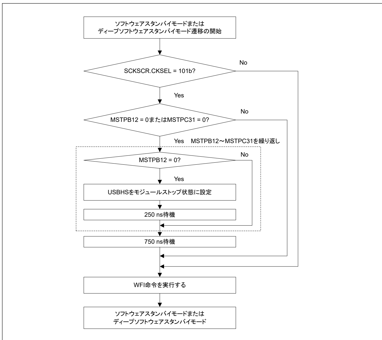
図 10.2 ソフトウェアスタンバイモードまたはディープソフトウェアスタンバイモード遷移時のフローチャート例
