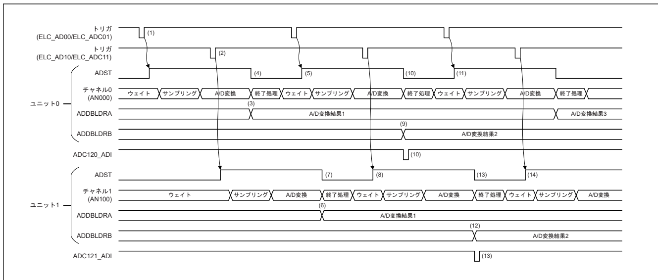
図 43.27 シングルスキャンモードの動作例（ダブルトリガ拡張モード選択、AN000 および AN100 選択、インターリーブ動作）
