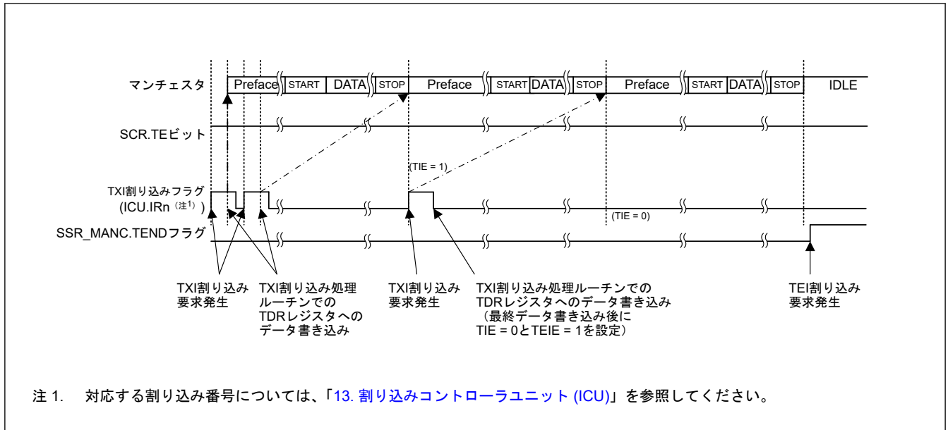
図 30.58 マンチェスタモードにおけるシリアル送信の終了動作の例（プレフィスあり、CTS 機能なし）
