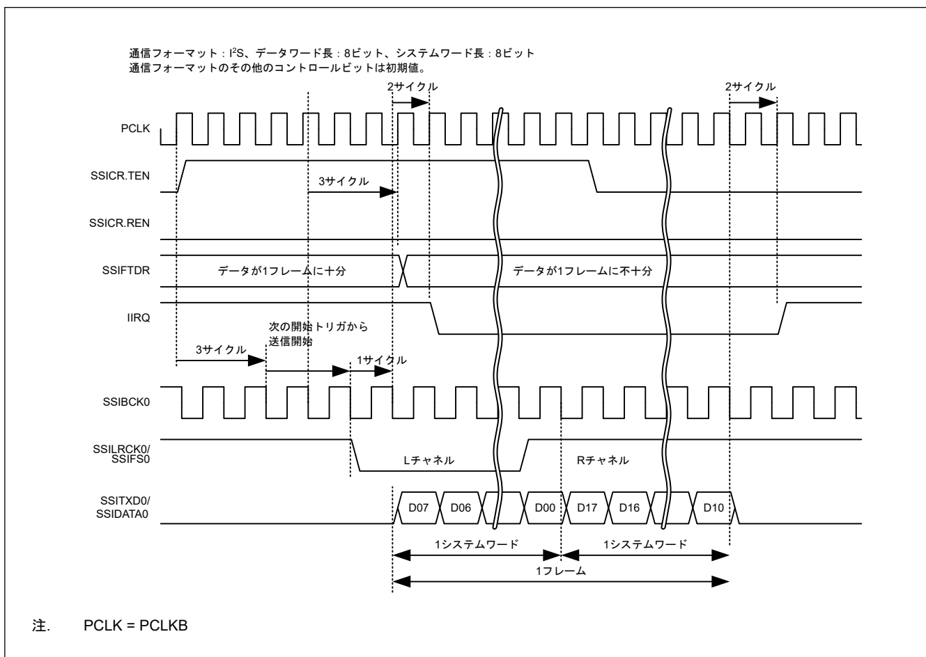
図 38.14 IIRQ 設定タイミング (送信)
