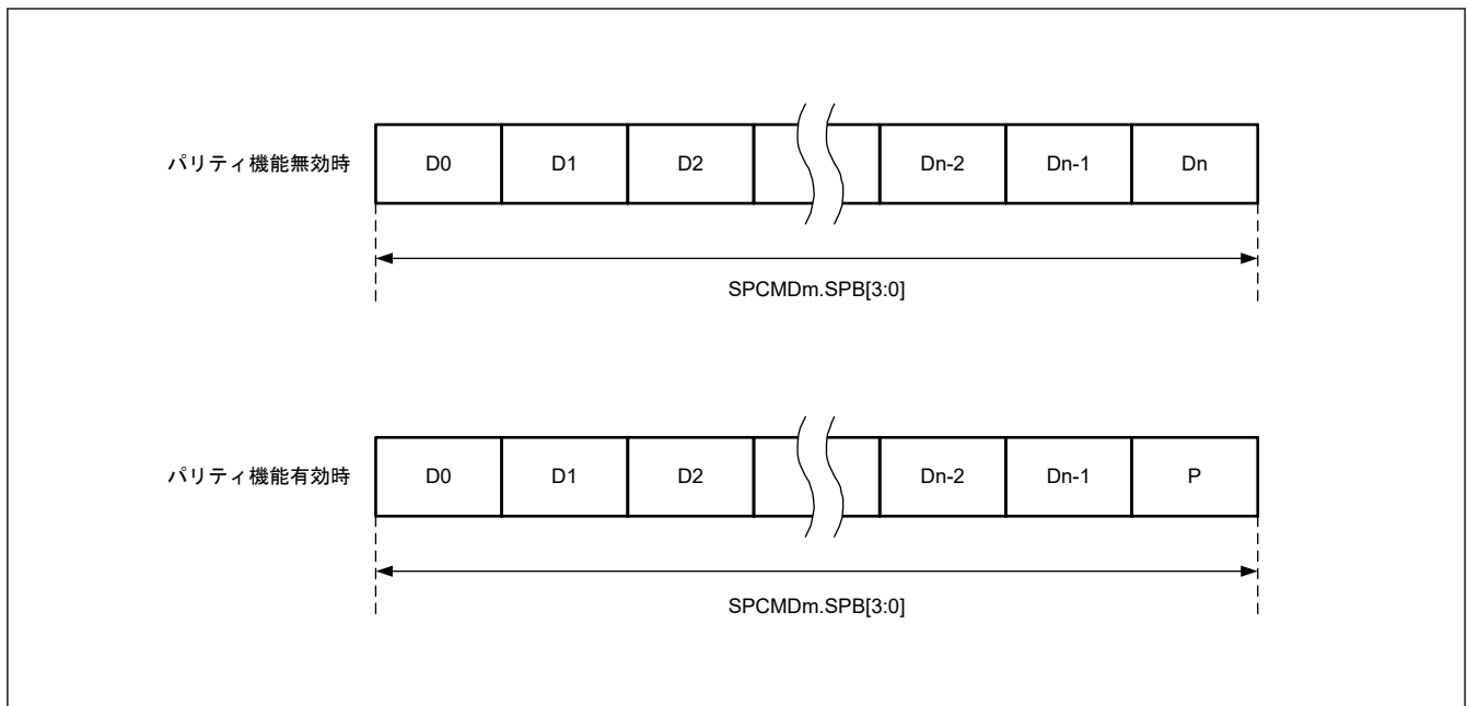
図 34.13 パリティ機能無効時と有効時のデータフォーマット
