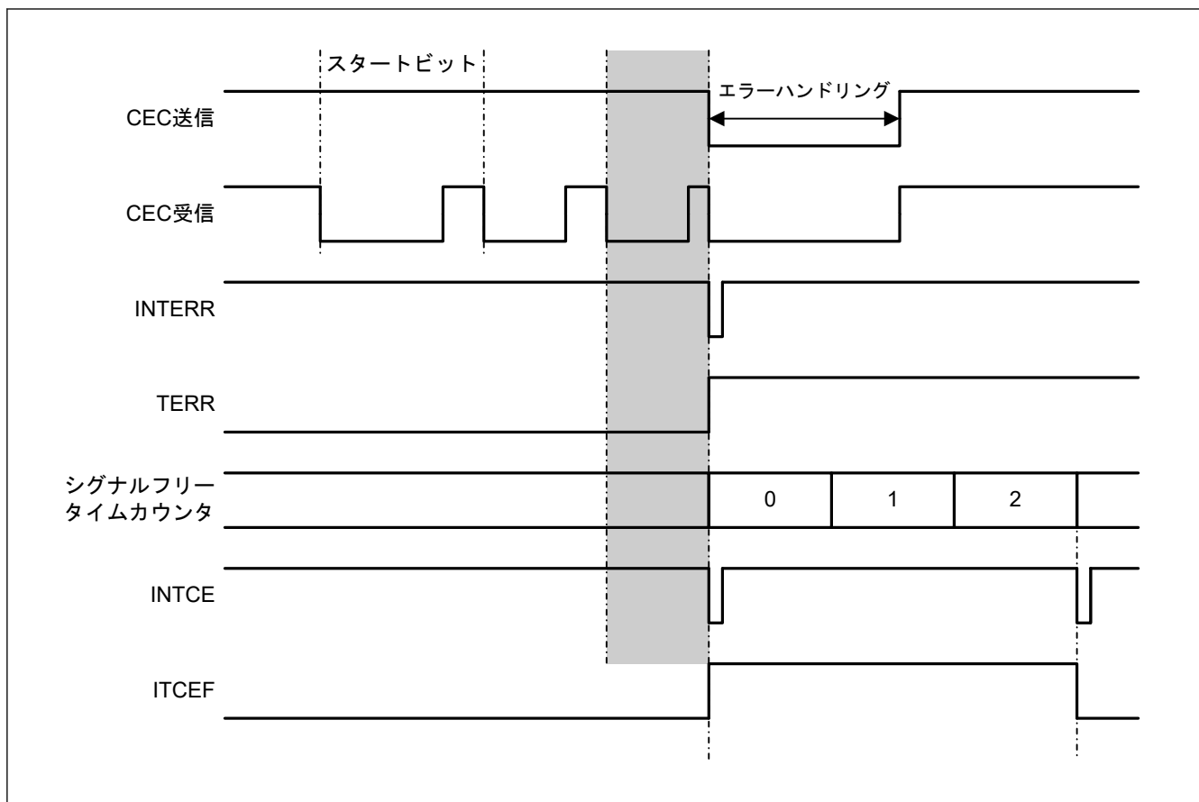
図 37.41 フォロワー動作時のビット幅が短い場合のタイミングエラー
