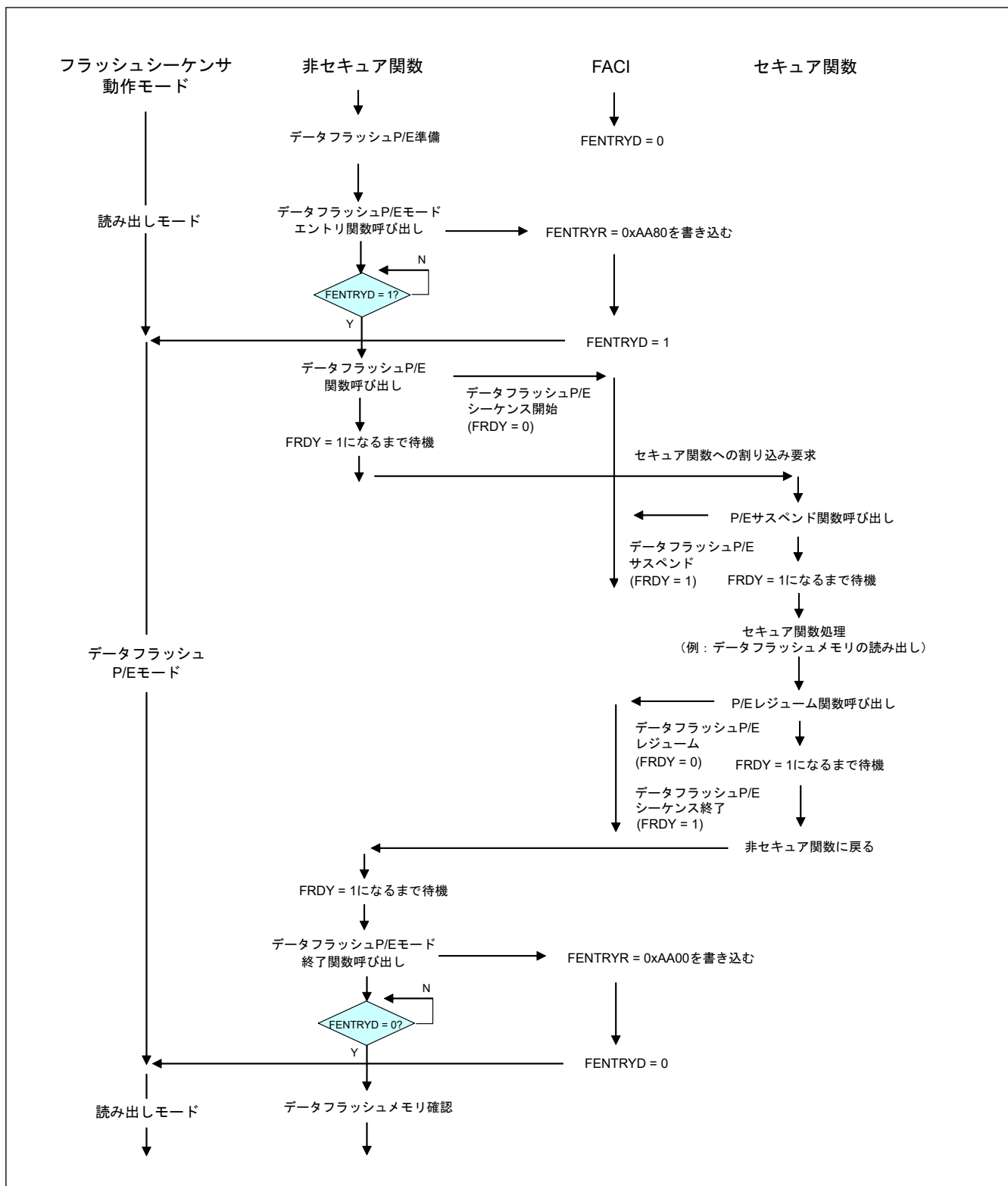
図 50.40 セキュア関数のデータフラッシュ P/E サスペンド例 (P/E 終了を検出するには FRDY ビットを確認)
