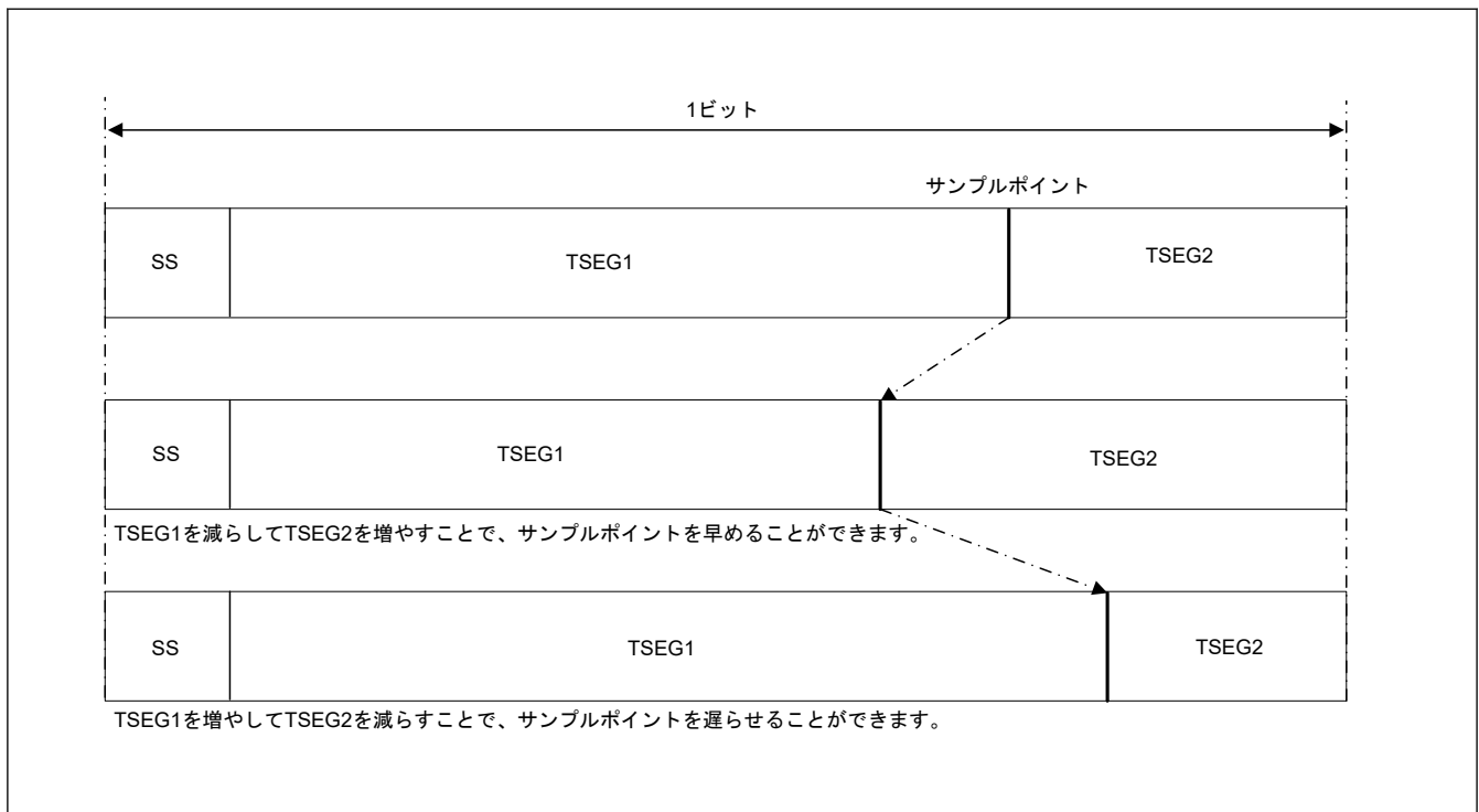
図 32.15 ビット内のセグメント構成とサンプルポイント
