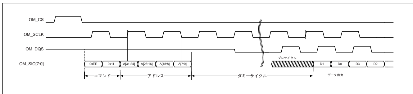
図 36.9 OctaFlash インタフェースでの読み出し動作の波形 (プレサイクル許可を使用した DOPI モード)
