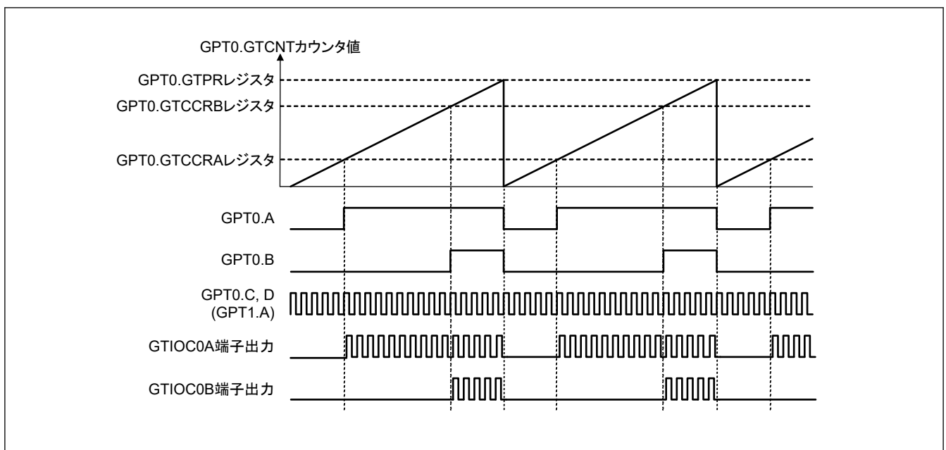
図 21.62 チャンネル間論理演算の例
