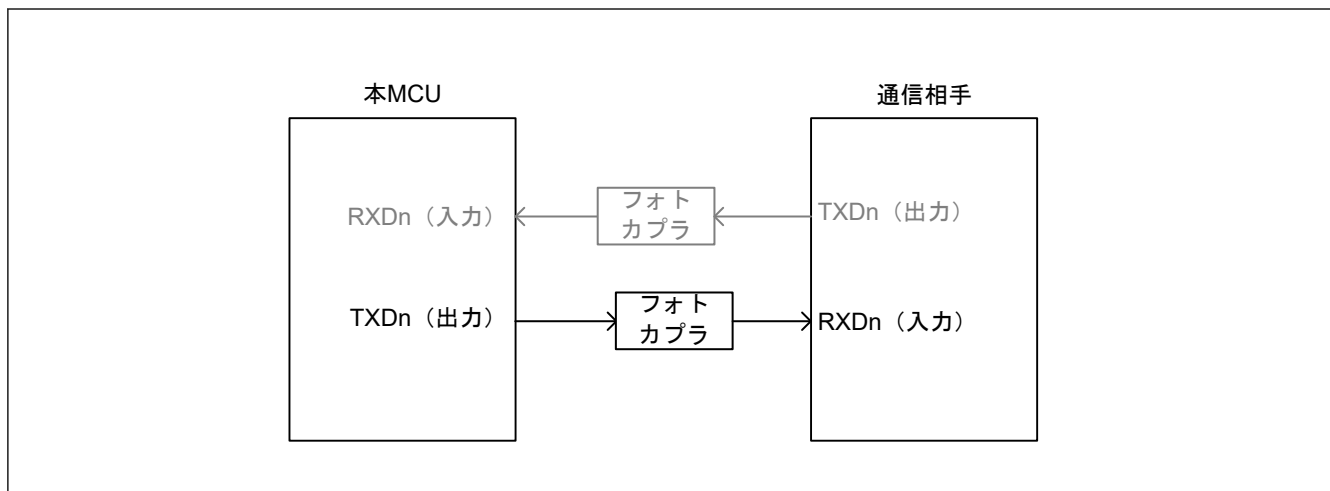
図 30.35 フォトカプラを通過する送信のブロック図イメージ
