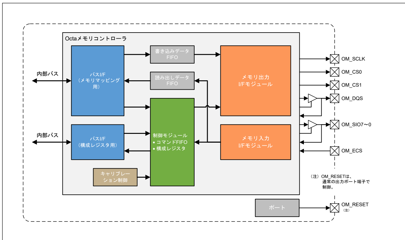
図 36.1 ブロック図
