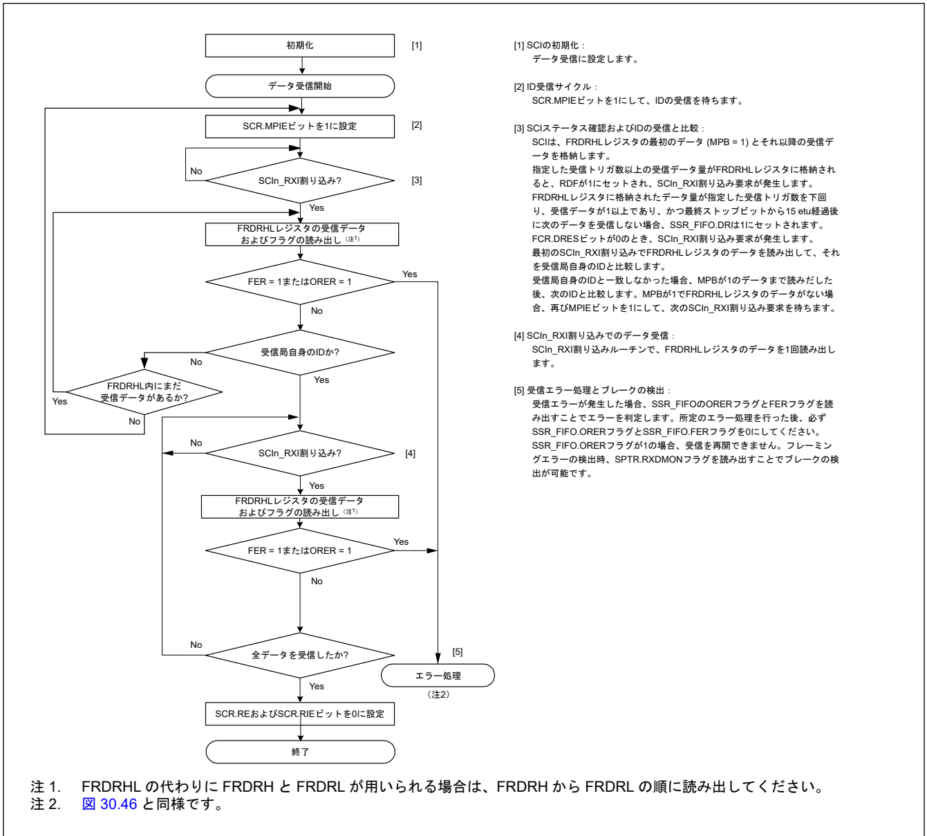
図 30.48 マルチプロセッサモードにおけるシリアル受信のフローチャート例 (FIFO 選択時)
