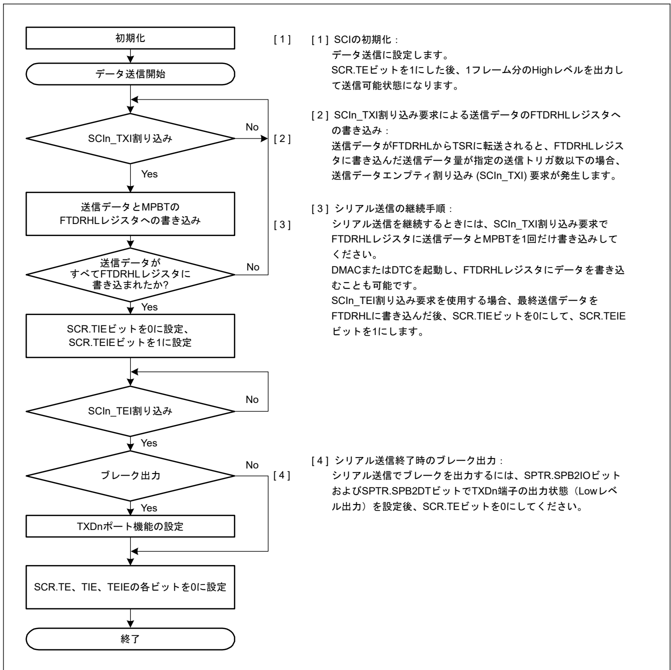
図 30.43 マルチプロセッサモードにおけるシリアル送信のフローチャート例 (FIFO 選択時)
