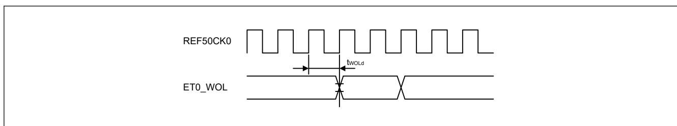
図 53.68 RMIi に対する WOL 出力タイミング
