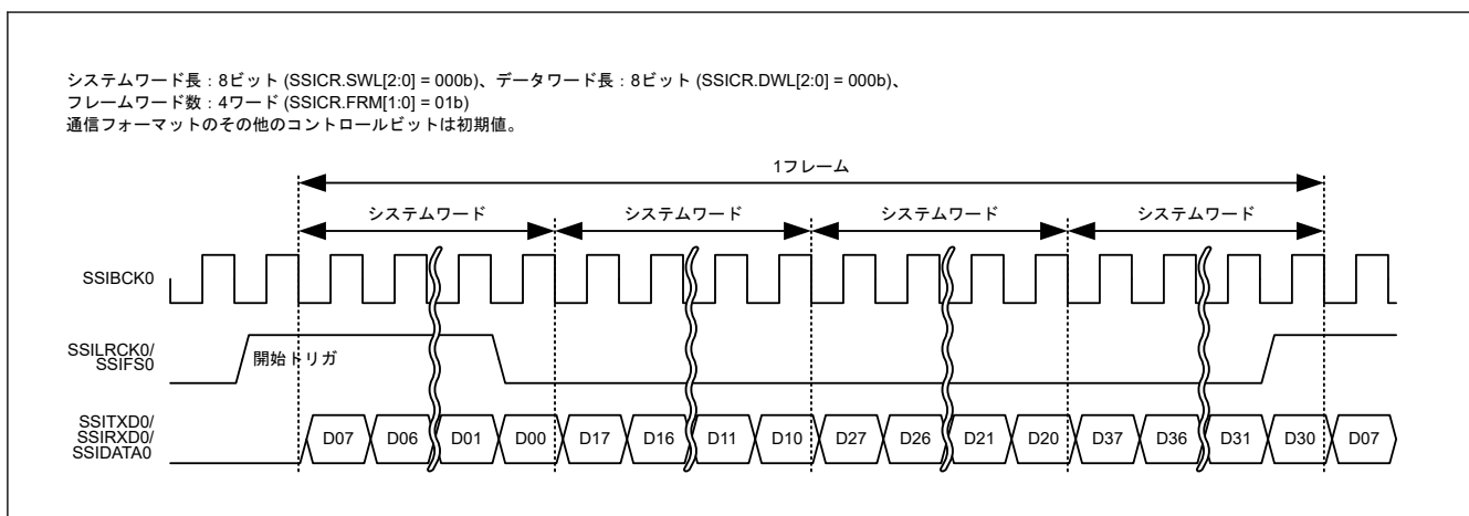
図 38.41 TDM フォーマット (パディングなし、システムワード長 = データワード長)
