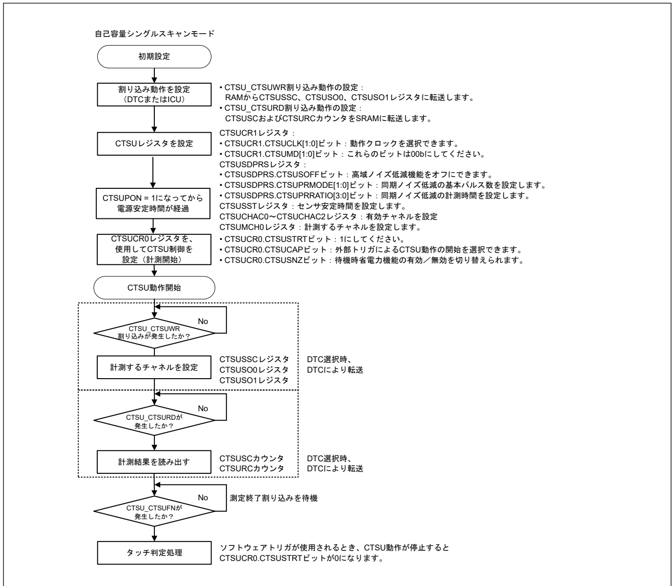
図 46.12 自己容量シングルスキャンモードのソフトウェアフローと動作例
