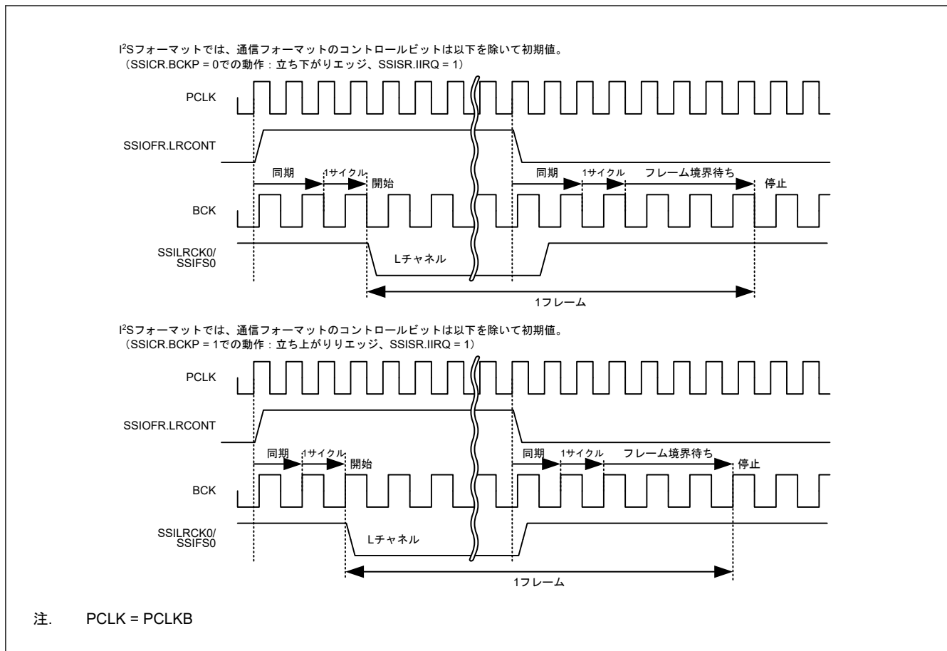
図 38.44 SSIOFR.LRCONT による LR クロック/フレーム同期継続禁止の例
