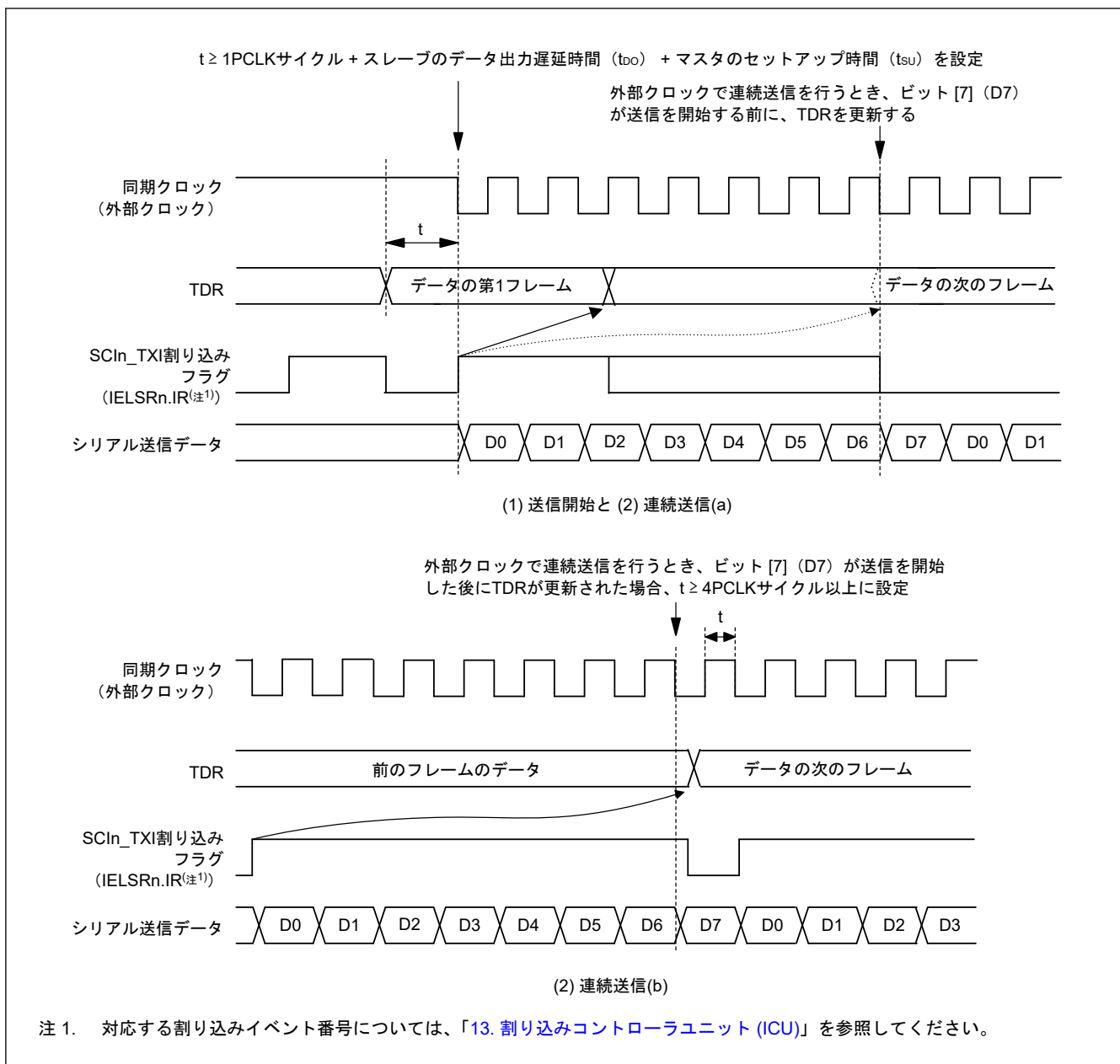
図 30.123 クロック同期式送信時の外部クロック使用に関する制約事項
