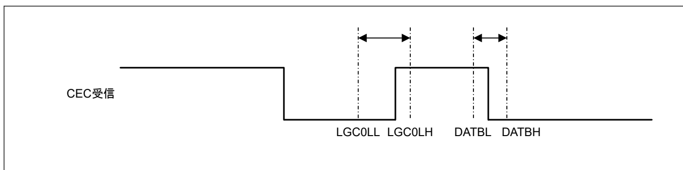
図 37.13 データビット (ロジカル 0) の受信タイミング
