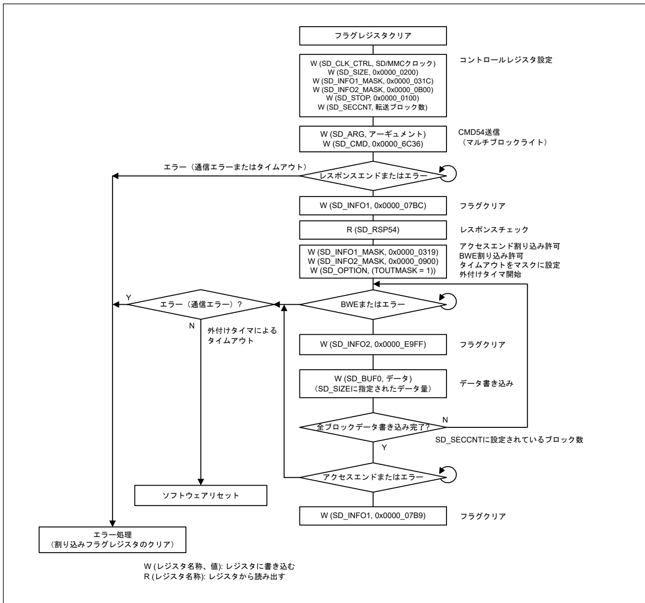
図 39.15 外付けタイマによるマルチブロックライト動作の例
