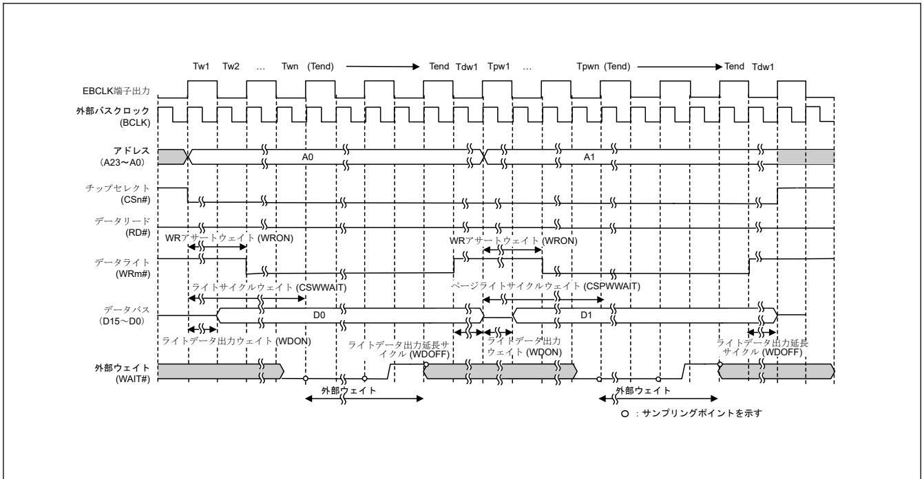
図 14.29 バイトストロープモード時の16ビットバス空間に対するページライトアクセスの外部ウェイトタイミング例 (EBCLK 端子出力選択ビットで BCLK の2分周を選択した場合) (n = 0~7, m = 0, 1)
