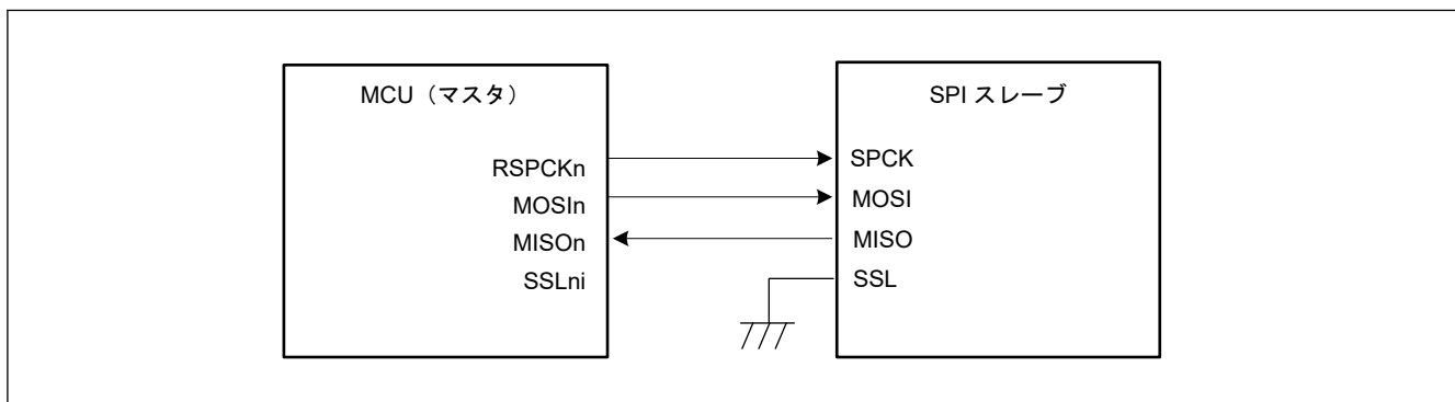
図 34.5 シングルマスタとシングルスレーブの構成例 (MCU はマスタ)
