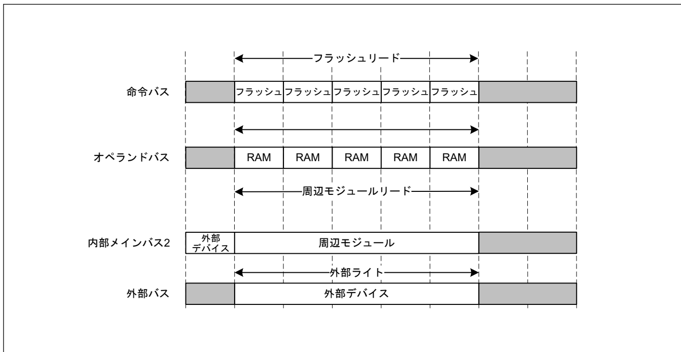
図 14.37 ライトバッファ機能使用時の動作例
