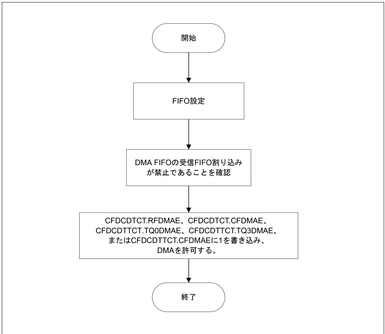
図 32.33 DMA 許可フロー
