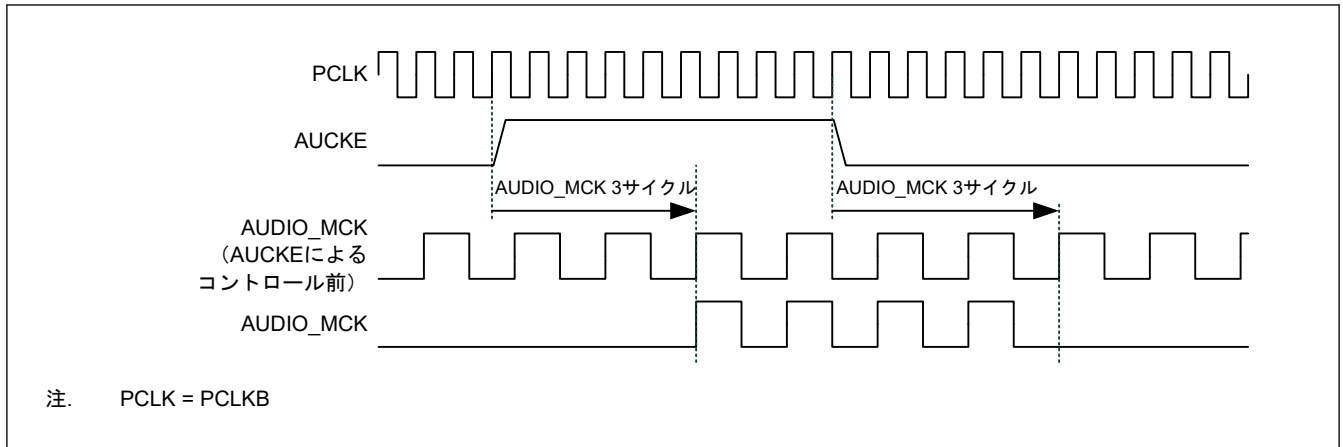
図 38.25 AUDIO_MCK の停止/再開
