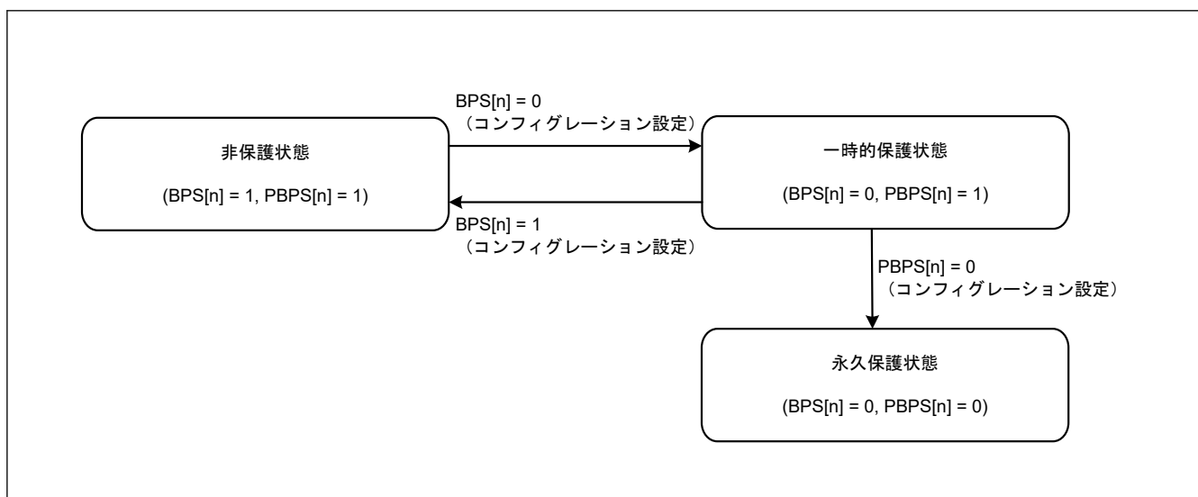
図 50.34 BPS[n]ビットおよび PBPS[n]ビットによるフラッシュシーケンサの状態遷移
