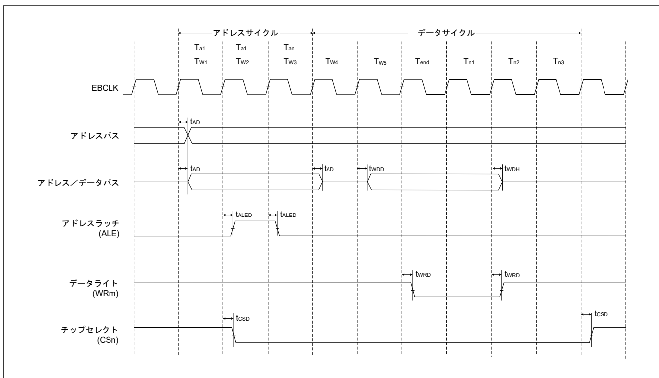
図 53.21 アドレス/データマルチプレクスバスのライトアクセスタイミング
