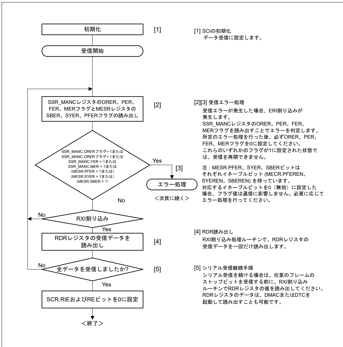
図 30.61 マンチェスタモードにおけるシリアルデータ受信フローチャートの例（正常受信）
