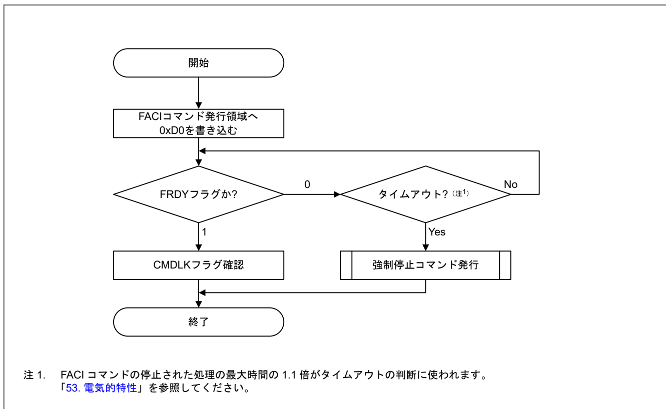
図 50.21 P/E レジュームコマンドの使用フロー
