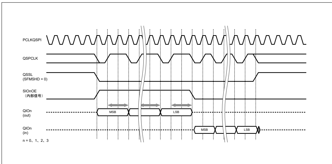
図 35.16 SFMOHW ビットを使用したシリアルデータ出力のホールド時間調整
