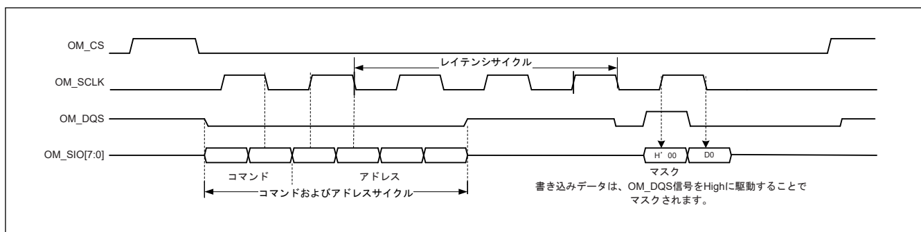
図 36.13 バイトマスクを許可した場合の書き込み動作の波形
