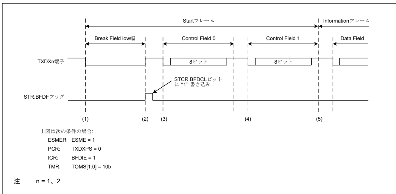
図 30.102 Start Frame 送信時の動作例
