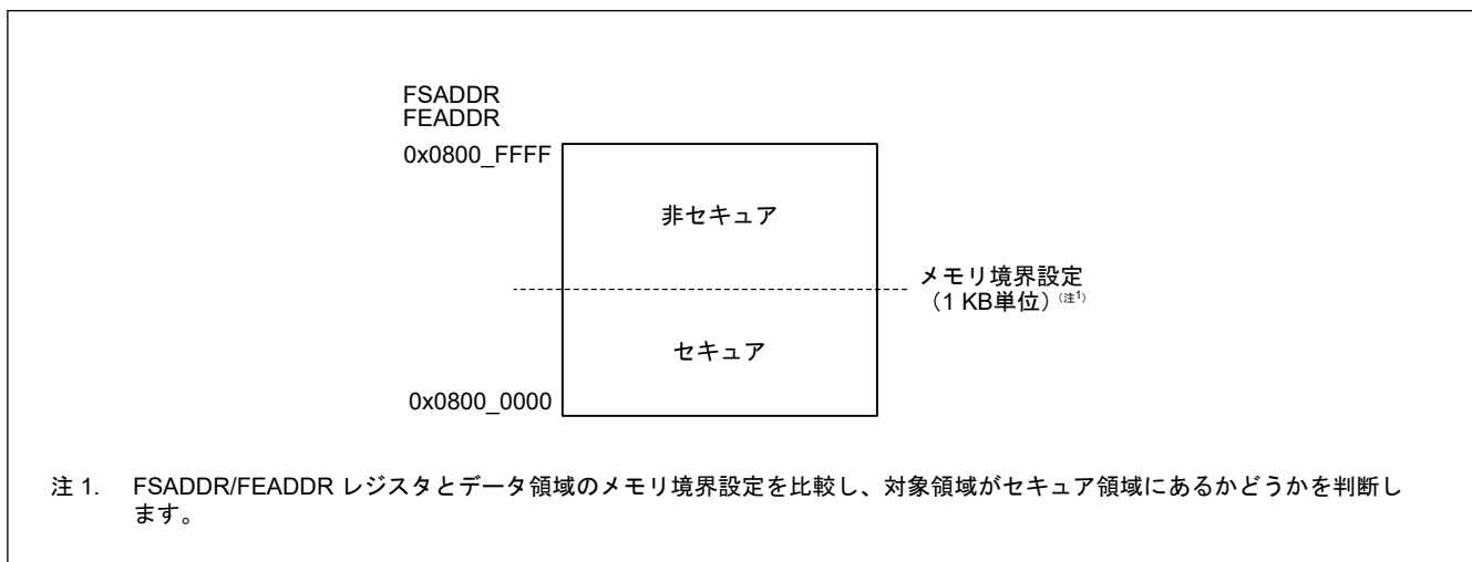
図 50.37 データ領域のセキュア/非セキュア領域
