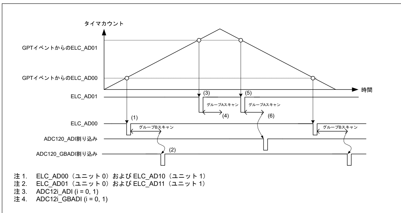
図 43.17 グループスキャンモードでダブルトリガモードを使用する場合の基本動作例 (ELC からの同期トリガ使用時)
