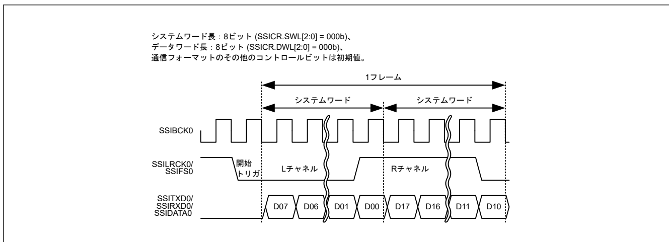
図 38.37 I 2 S フォーマット (パディングなし、システムワード長 = データワード長)
