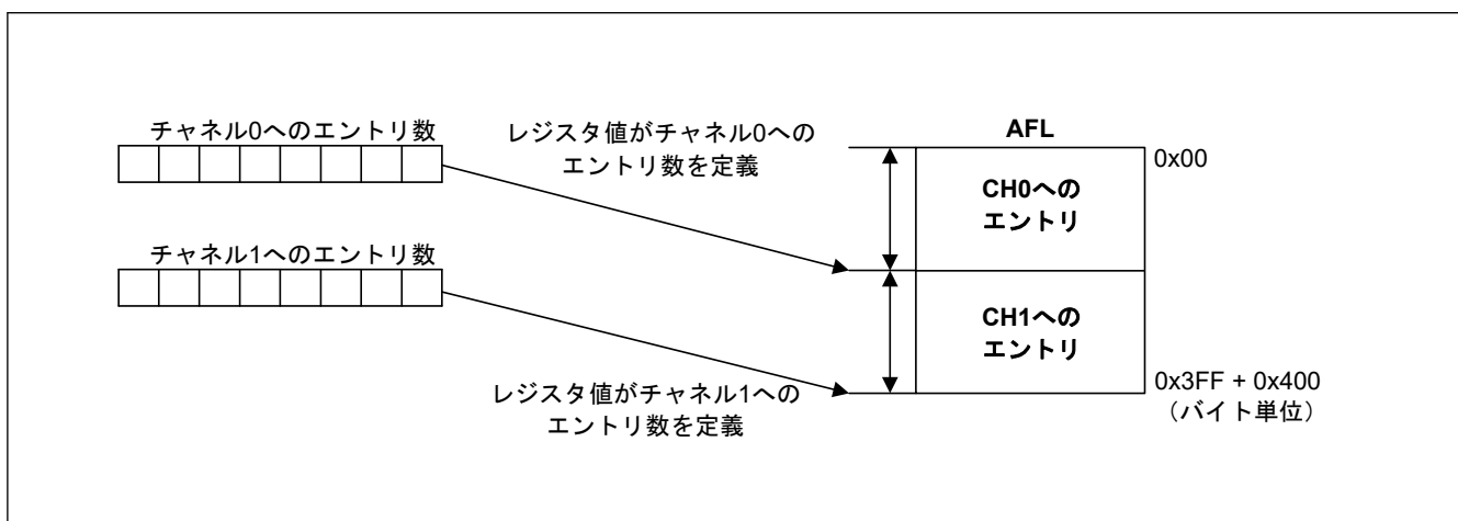
図 32.24 各チャンネルの AFL の構成
