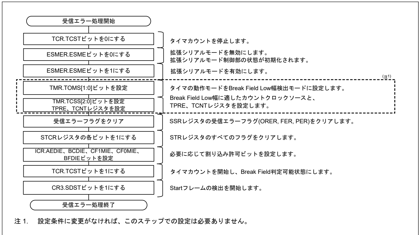
図 30.125 受信エラー処理のフローチャートの例 (スタートフレーム受信時)
