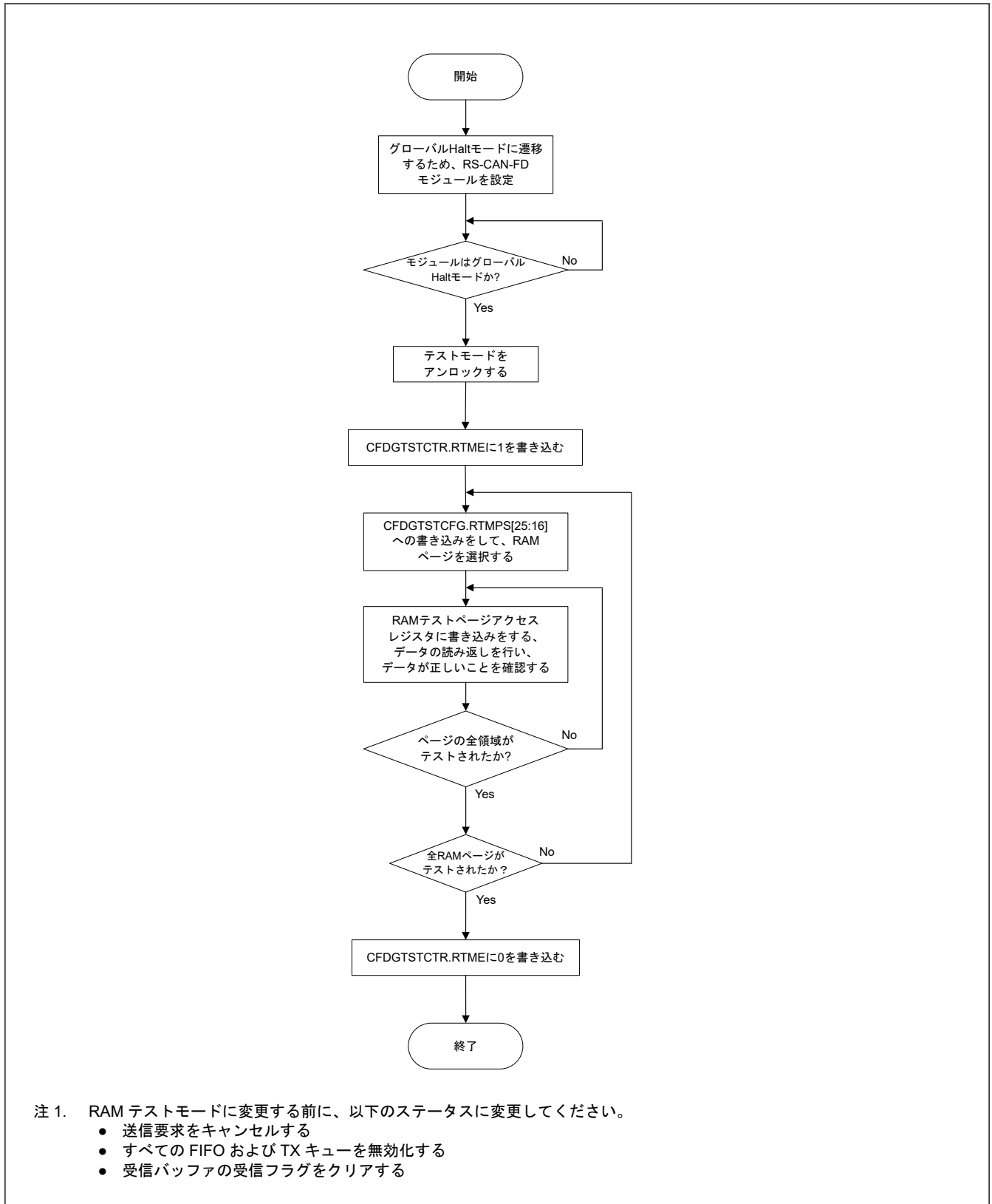
図 32.52 RAM テストモードのソフトウェアフロー
