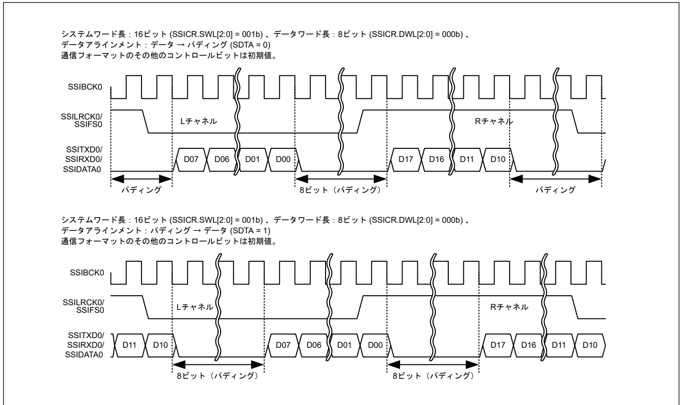
図 38.10 パディングビットを伴うシリアルデータのアライメント設定
