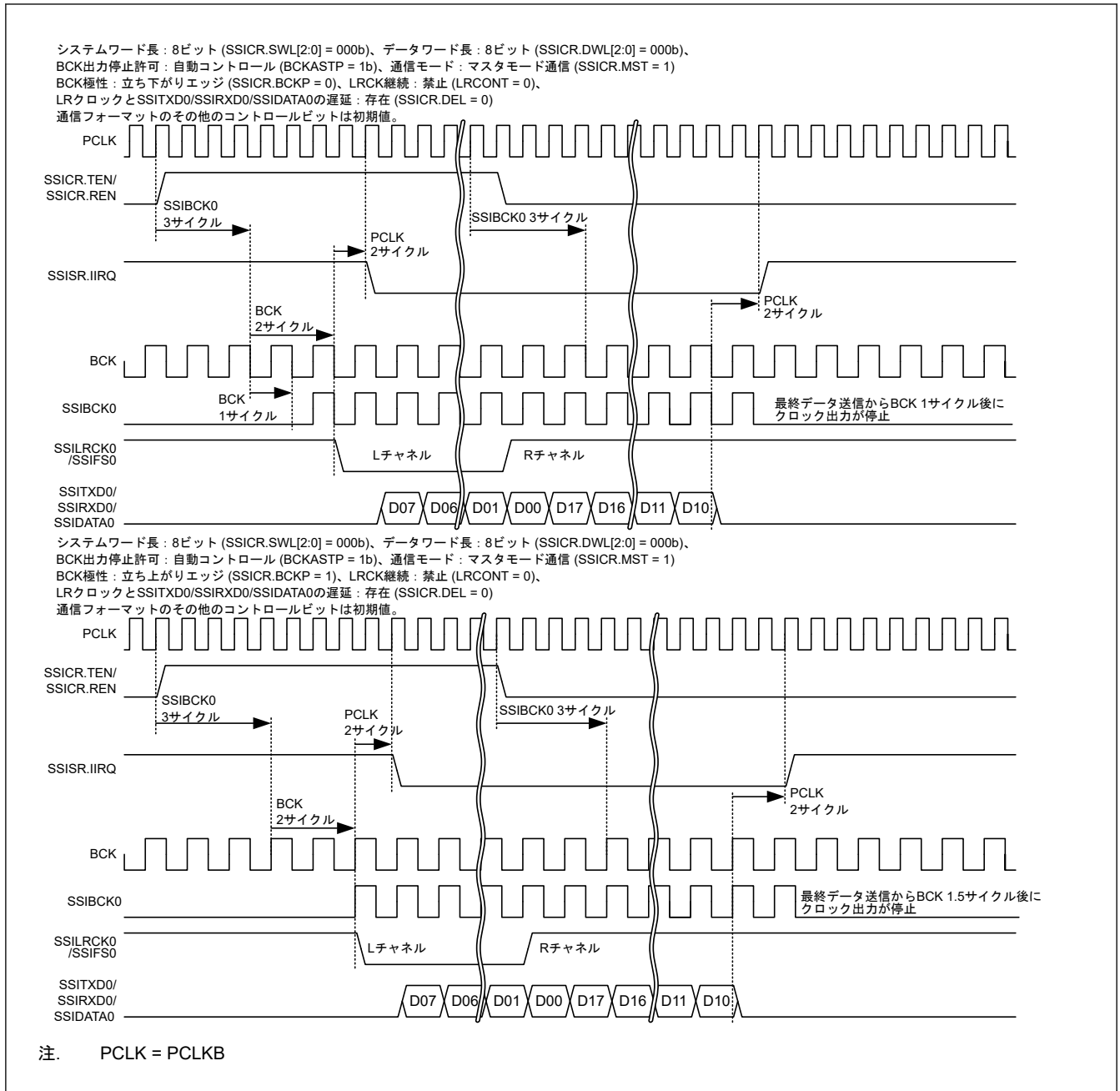
図 38.35 BCKASTP ビットの動作例 (BCKASTP = 1 での通信動作の場合)
