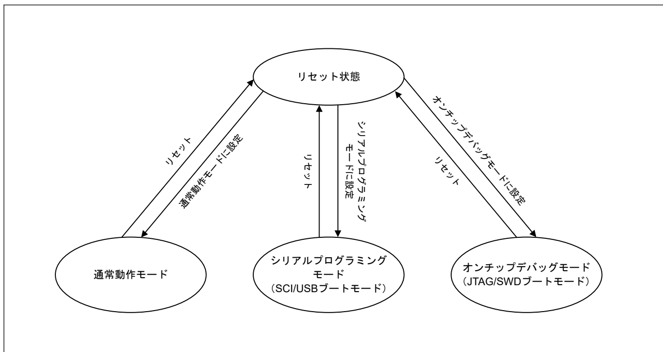
図 50.6 フラッシュメモリに関するモード遷移図
