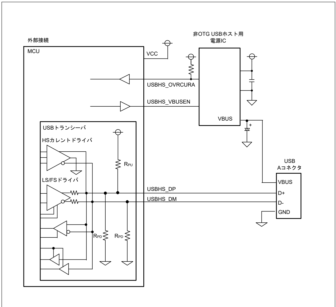
図 29.30 USB ホスト接続例
