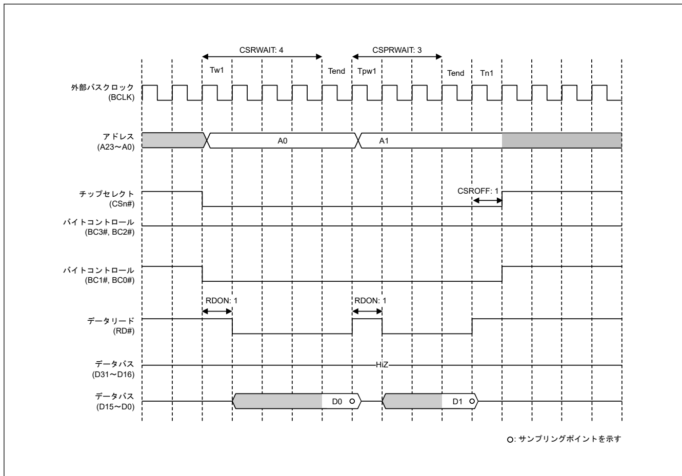
図 14.19 ページリードアクセスの動作例 (16 ビットバス空間に対する 32 ビットアクセスの場合) (n = 0~7)
