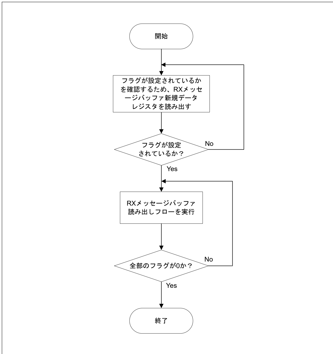
図 32.35 RX メッセージバッファのアクセス手順
