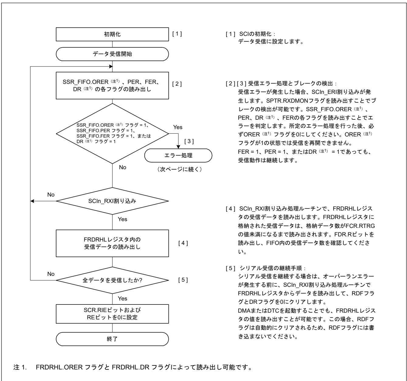
図 30.26 調歩同期式モードにおけるシリアル受信のフローチャート例 (FIFO 選択、アドレス一致検出有効時) (1)
