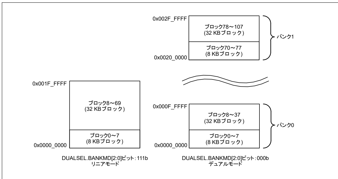
図 50.30 バンクモード切り替えフロー例 (2 M バイトのコードフラッシュメモリを持つ製品の場合)
