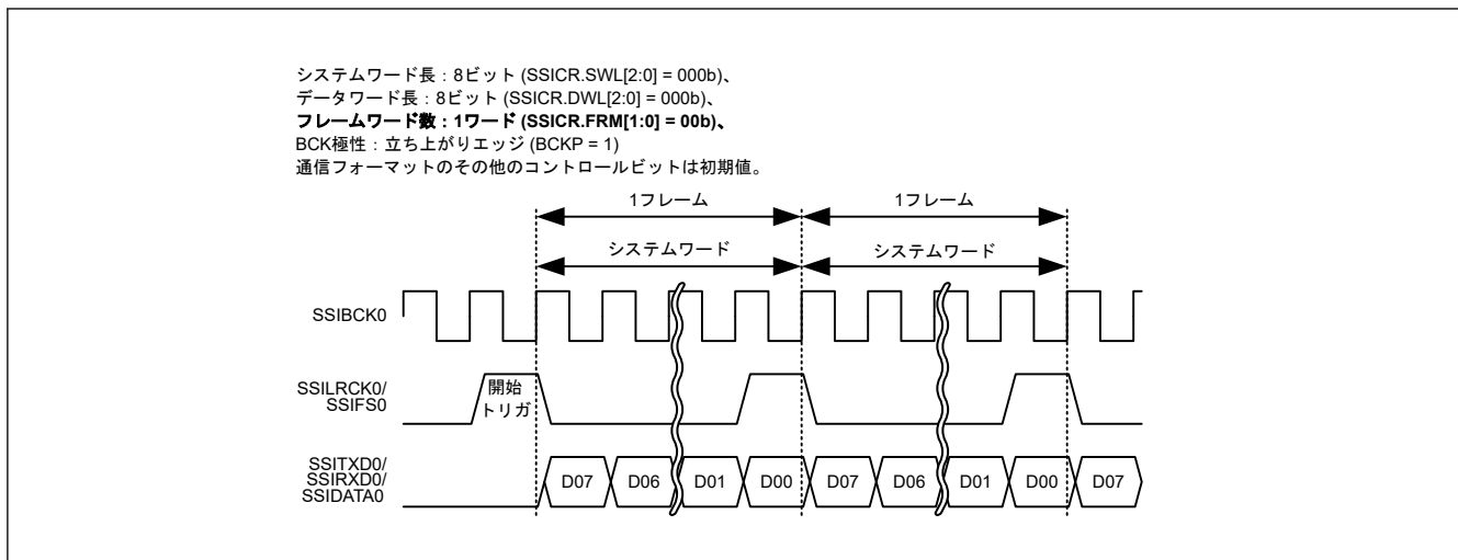
図 38.38 モノラルフォーマットにおけるショートフレーム（パディングなし、システムワード長 = データワード長）
