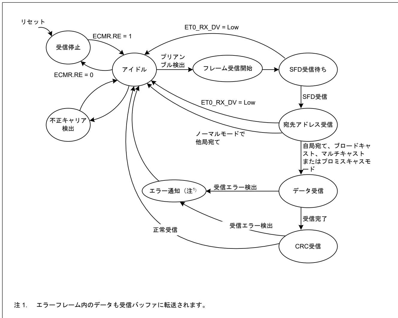
図 26.5 ETHERC 送信部の状態遷移
