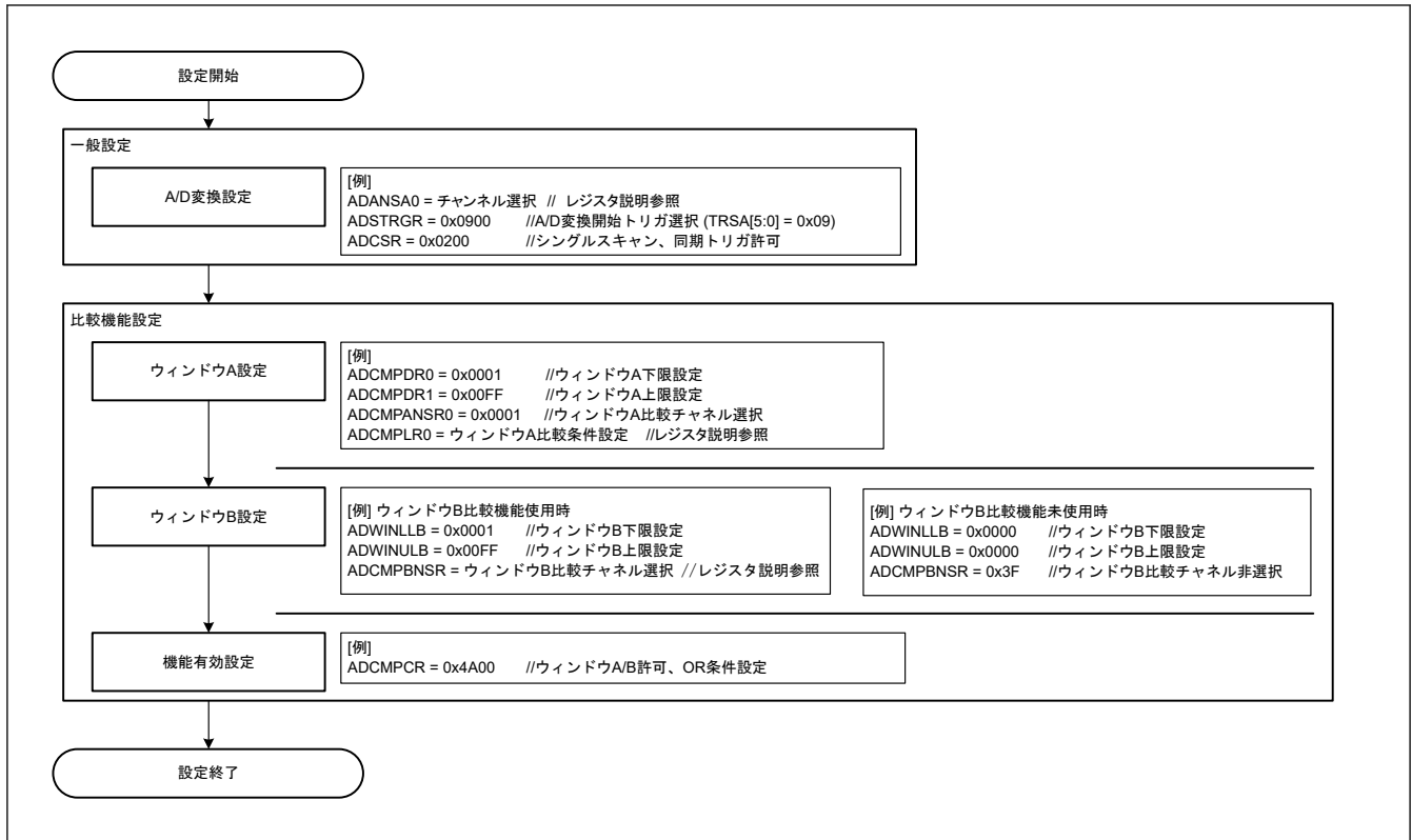
図 43.29 コンペア機能のイベント出力使用時の設定例
