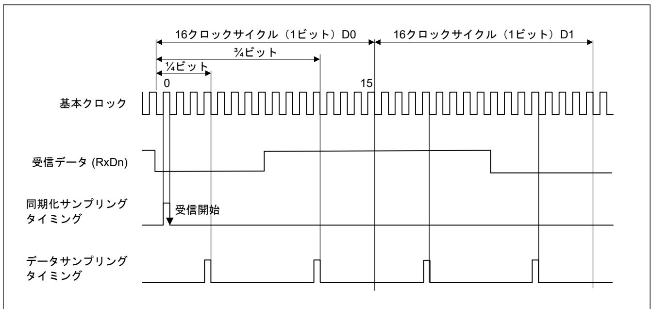
図 30.59 マンチェスタモードでのデータ受信サンプリングタイミング
