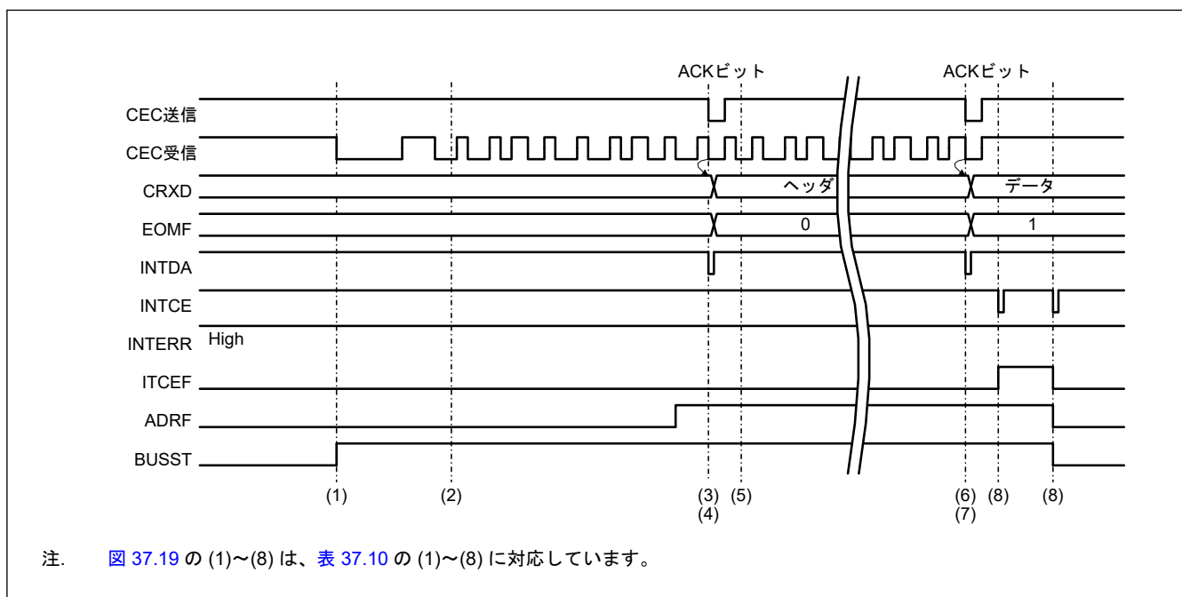
図 37.19 受信基本タイミング (1) (ダイレクトアドレス受信、CECCTL1.CESEL[1:0] = 00b のとき)
