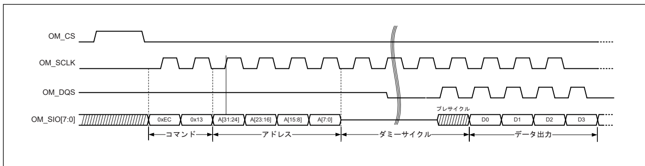
図 36.8 OctaFlash インタフェースでの読み出し動作の波形 (プレサイクル許可および DQS 許可を使用した SOPI モード)
