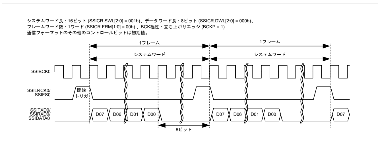
図 38.39 モノラルフォーマットにおけるショートフレーム（パディングあり、システムワード長 > データワード長）
