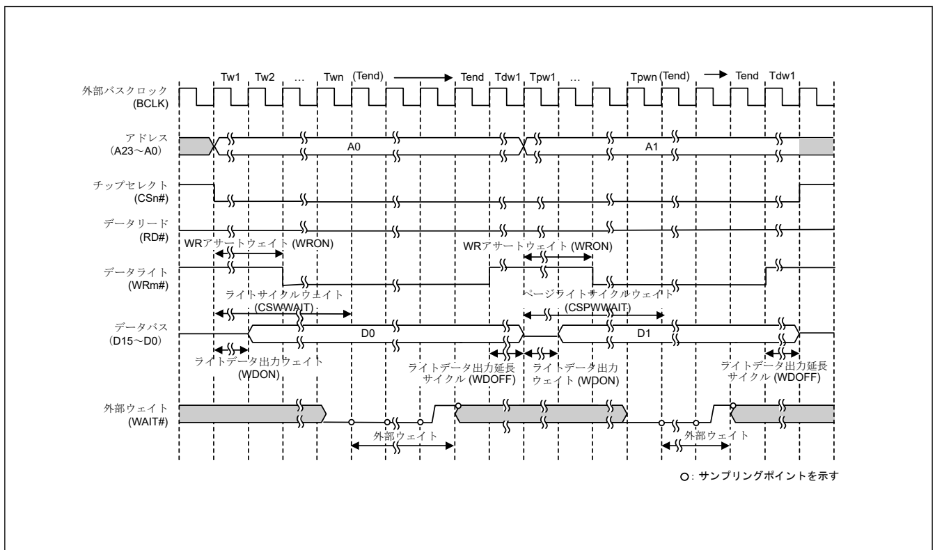
図 14.28 バイトストロブモード時の 16 ビットバス空間に対するページライトアクセスの外部ウェイトタイミング例 (EBCLK 端子出力選択ビットで BCLK の 1 分周を選択した場合) (n = 0~7、m = 0、1)
