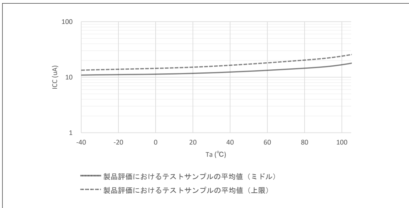
図 53.4 ディープソフトウェアスタンバイモード時の温度依存性、SRAM および USB レジューム検出部への電源供給なし、パワーオンリセット回路、低消費電力機能無効 (参考データ)
