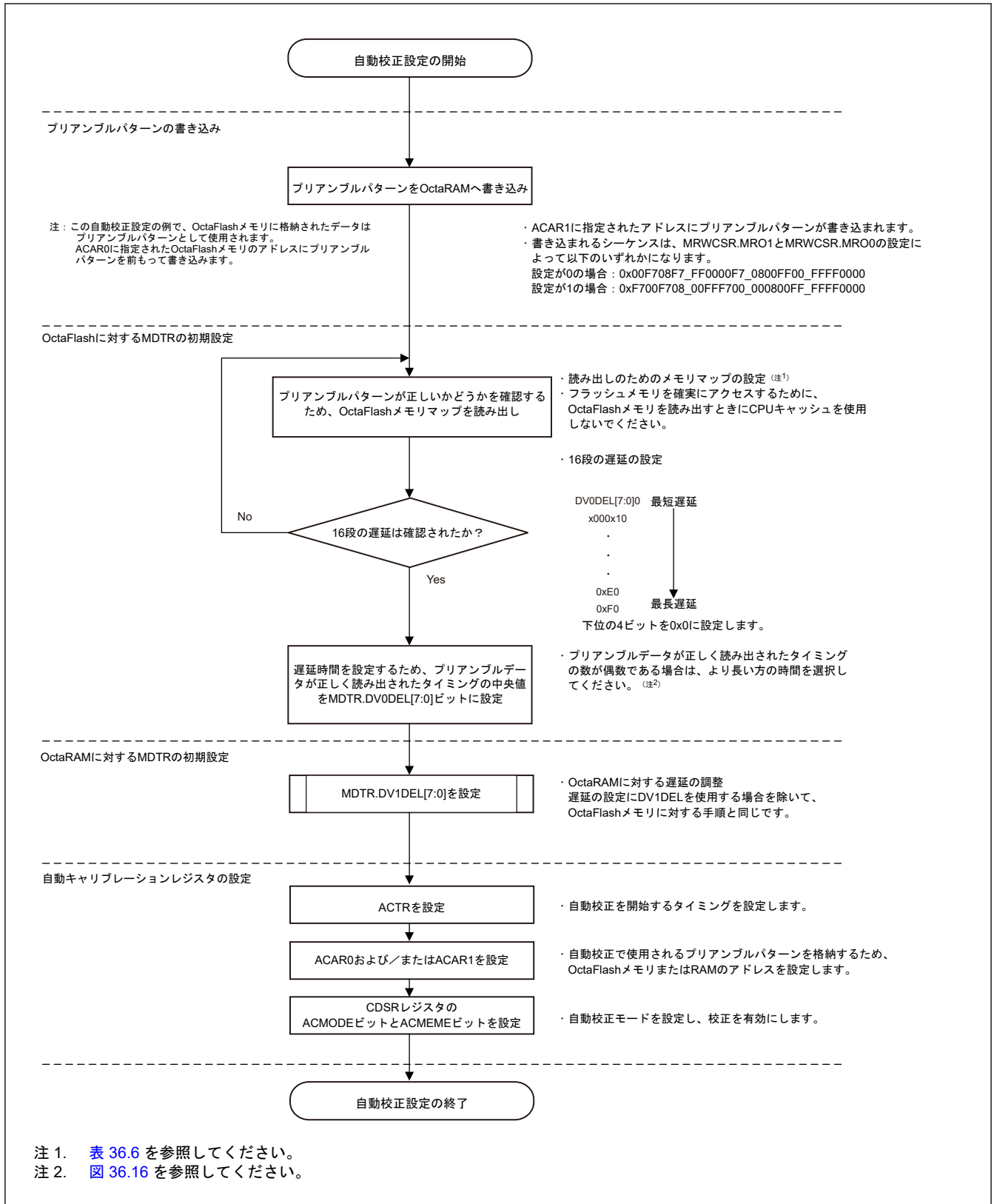
図 36.15 手動校正フローを用いた自動校正設定
