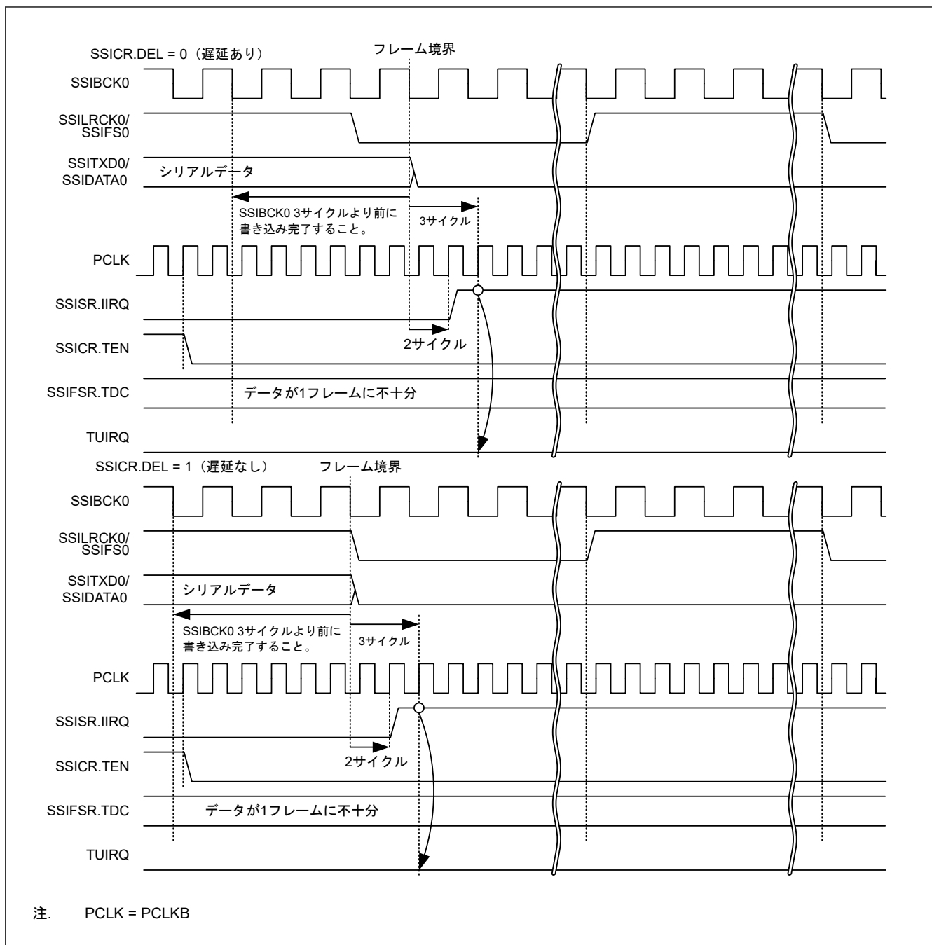
図 38.21 TUIRQ 設定タイミング (通信中断時)
