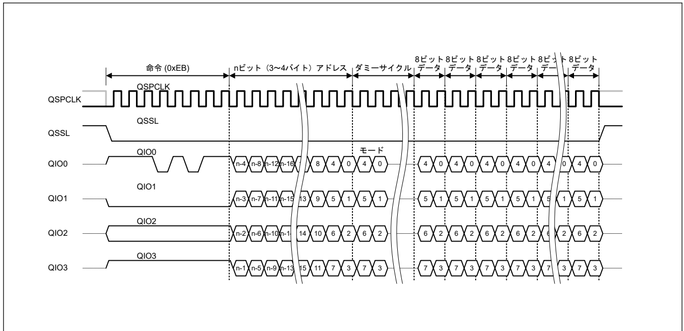
図 35.27 ファストリード Quad I/O パスサイクル
