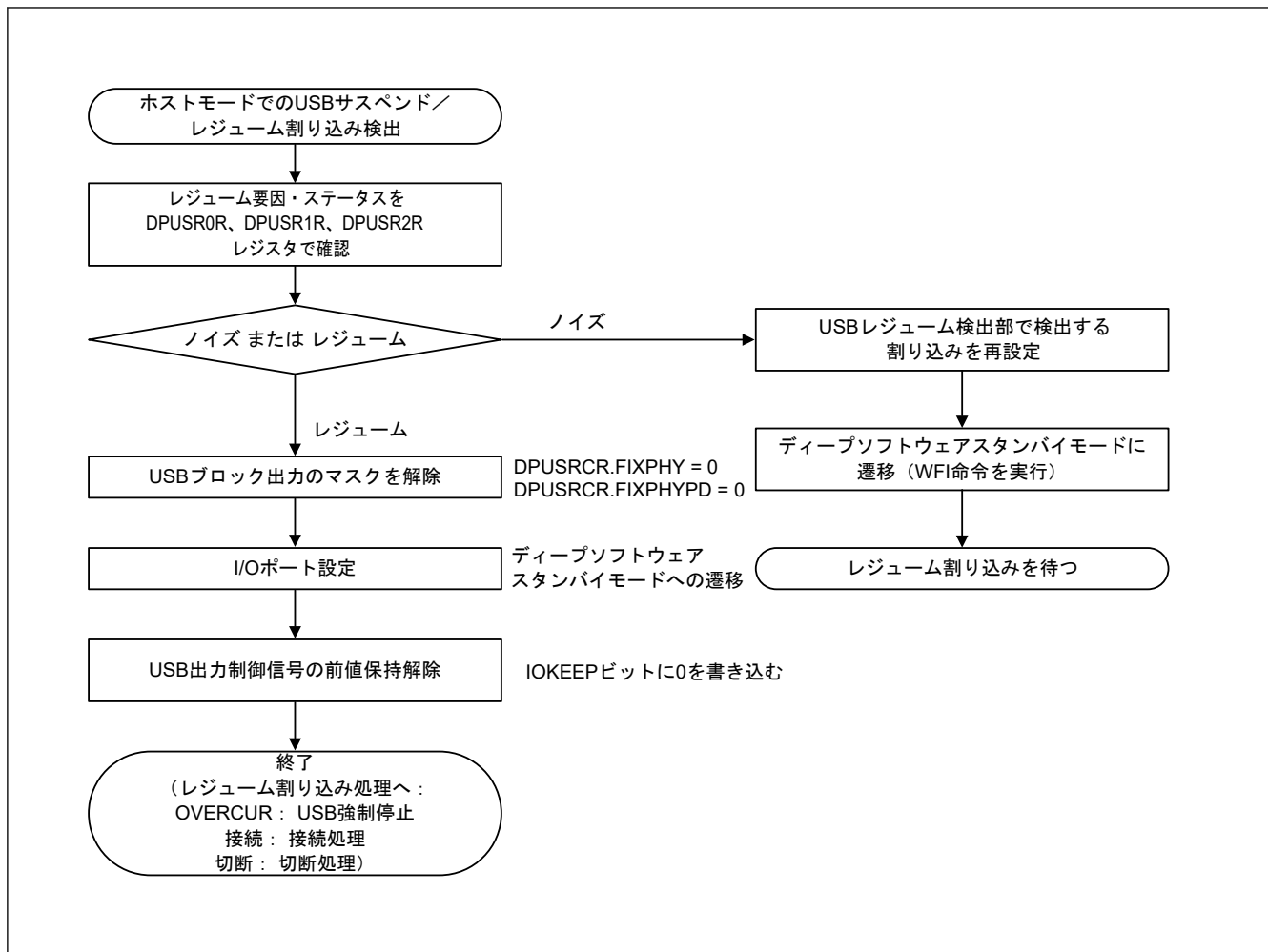
図 29.23 ホストコントローラとしてディープソフトウェアスタンバイモードを解除する場合の USBHS 設定フロー (1)
