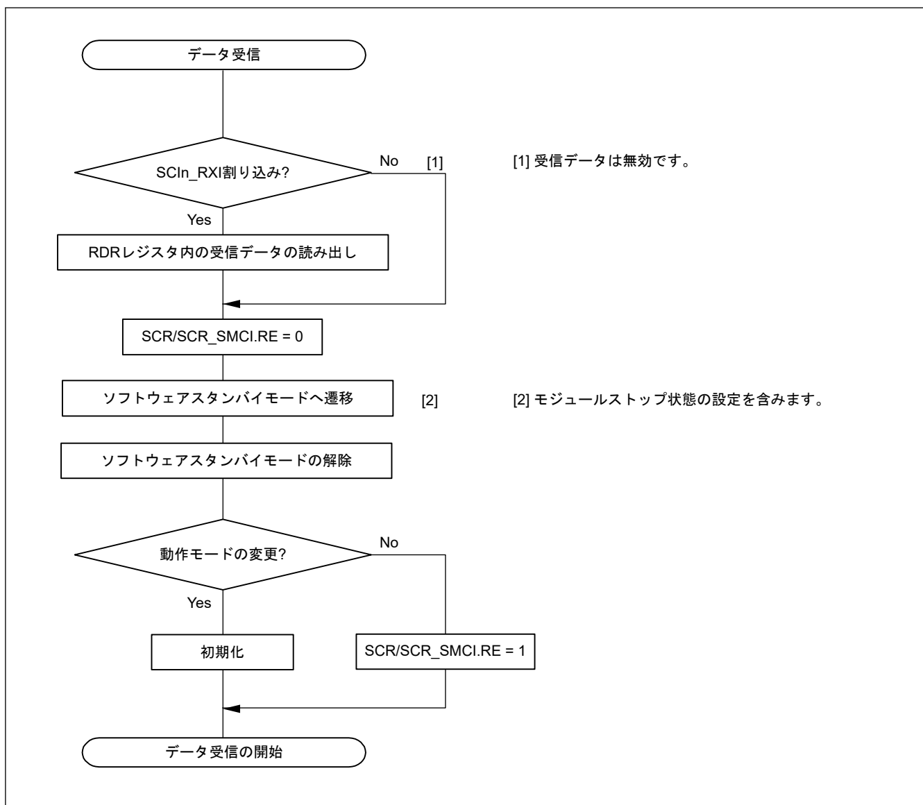
図 30.121 受信中にソフトウェアスタンバイモードへ遷移する場合のフローチャート例
