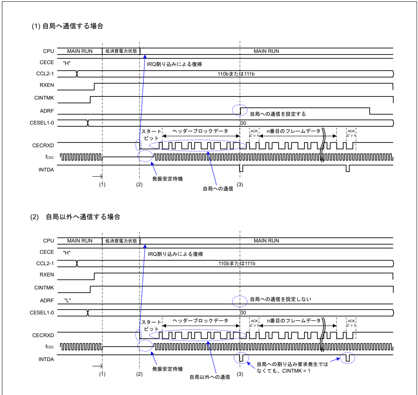
図 37.51 スタートビット立ち下がりエッジによる低消費電力状態からの復帰動作（自局判定）
