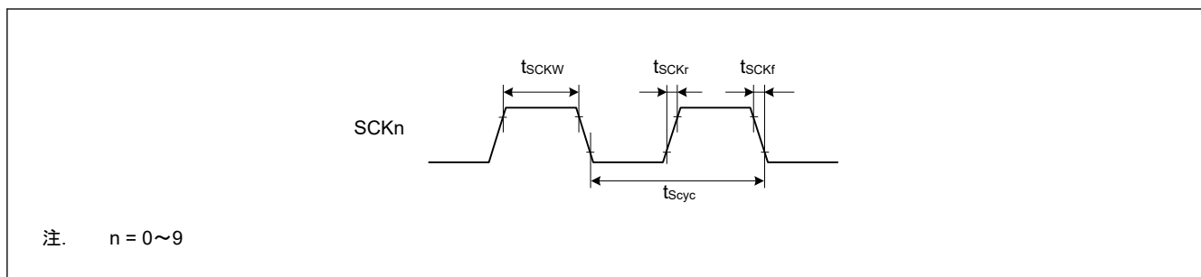
図 53.34 SCK クロック入出力タイミング
