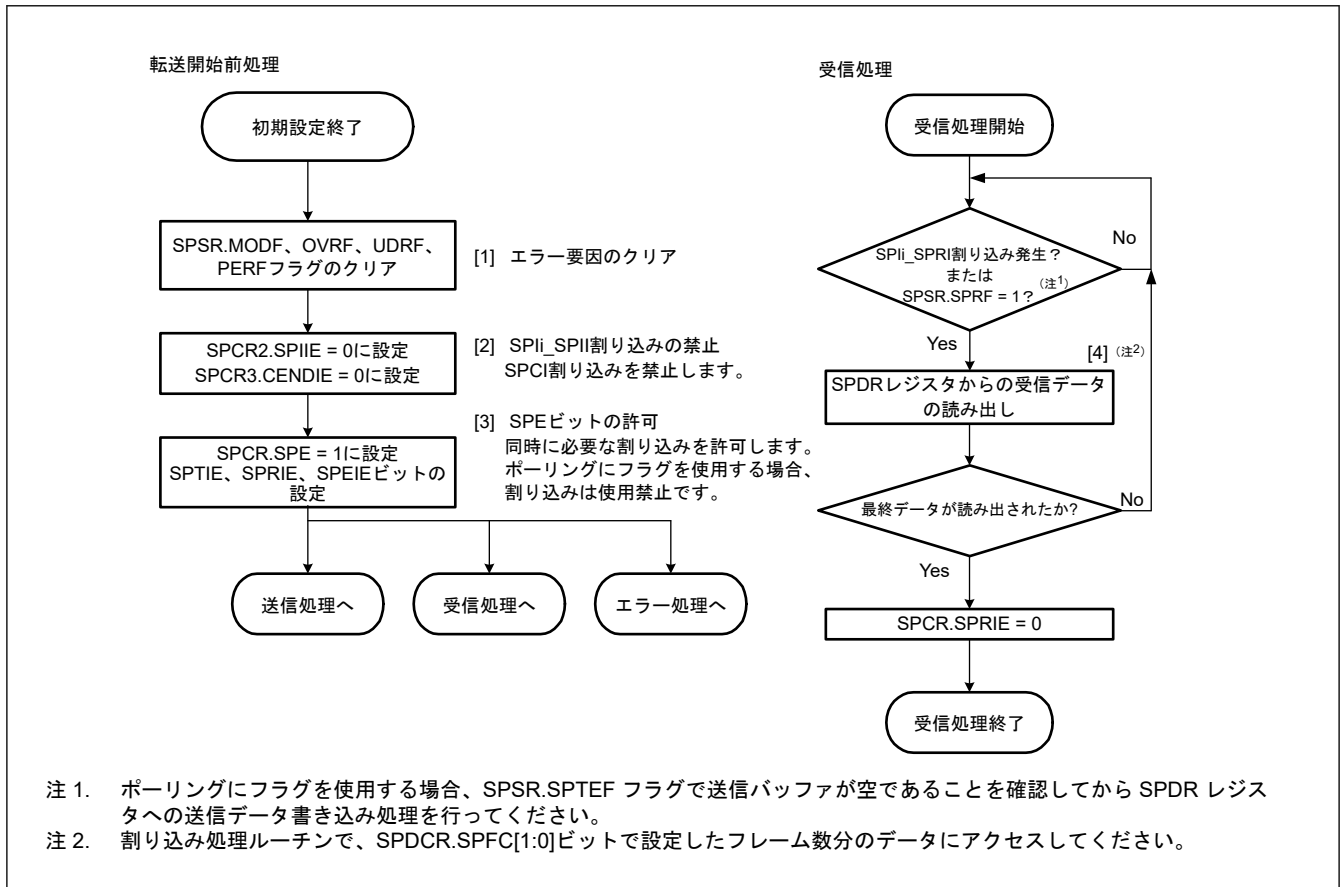
図 34.53 スレーブモードでの送信フロー
