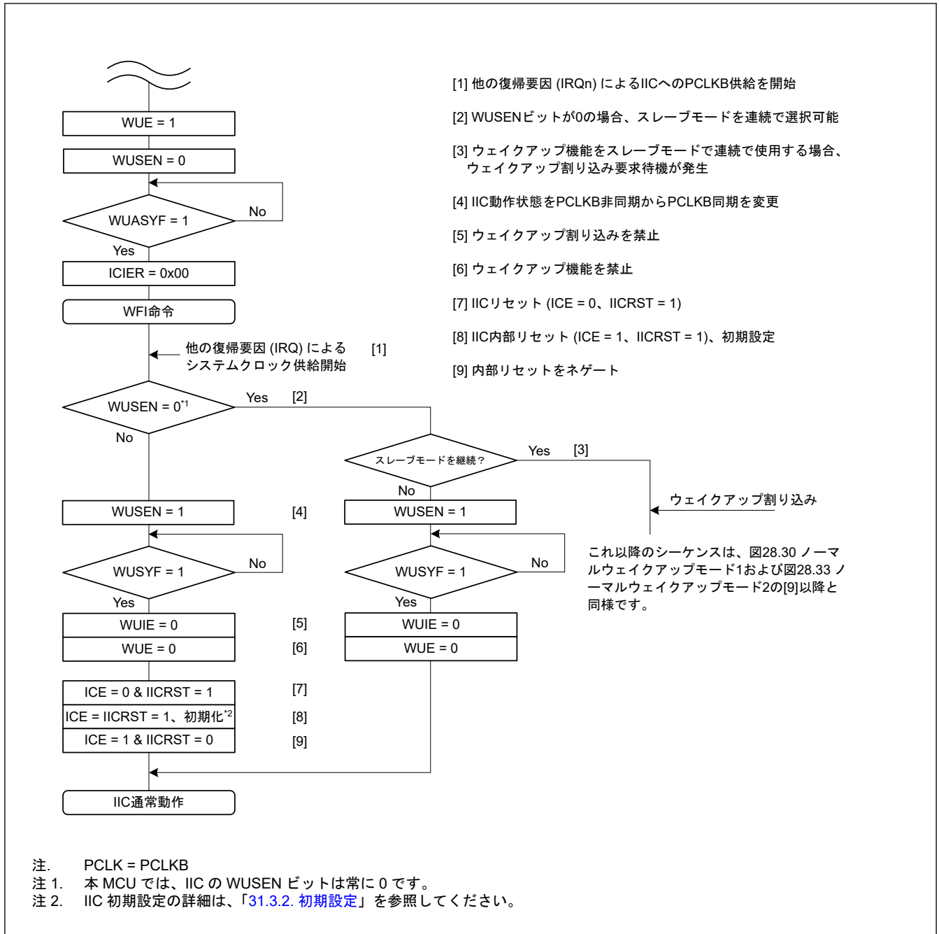
図 31.31 ノーマルウェイクアップモード1および2の動作例 (IIC ウェイクアップ割り込み以外の割り込み (たとえば IRQn) によるウェイクアップの場合)
