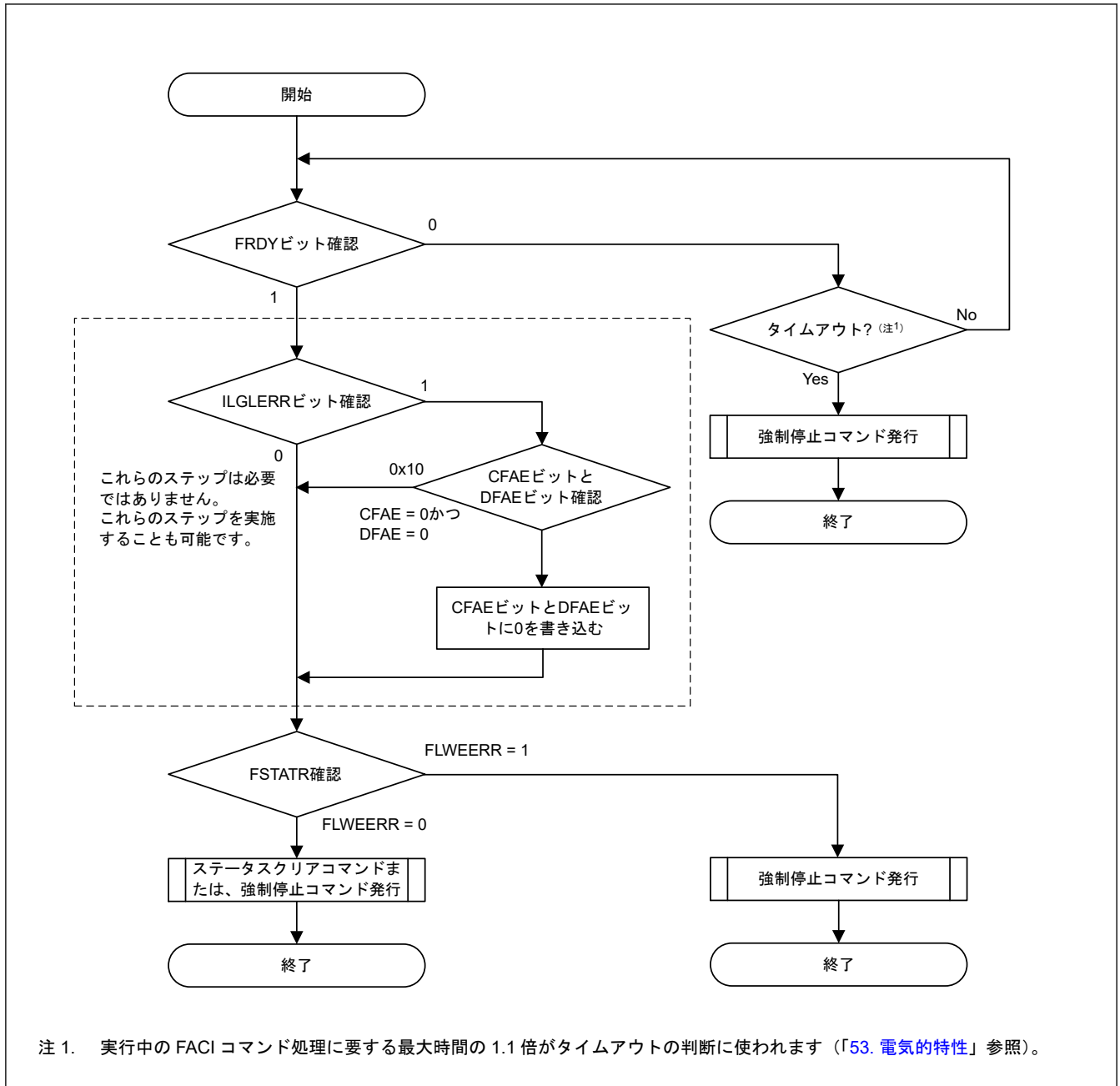
図 50.13 コマンドロック状態からの復帰フロー
