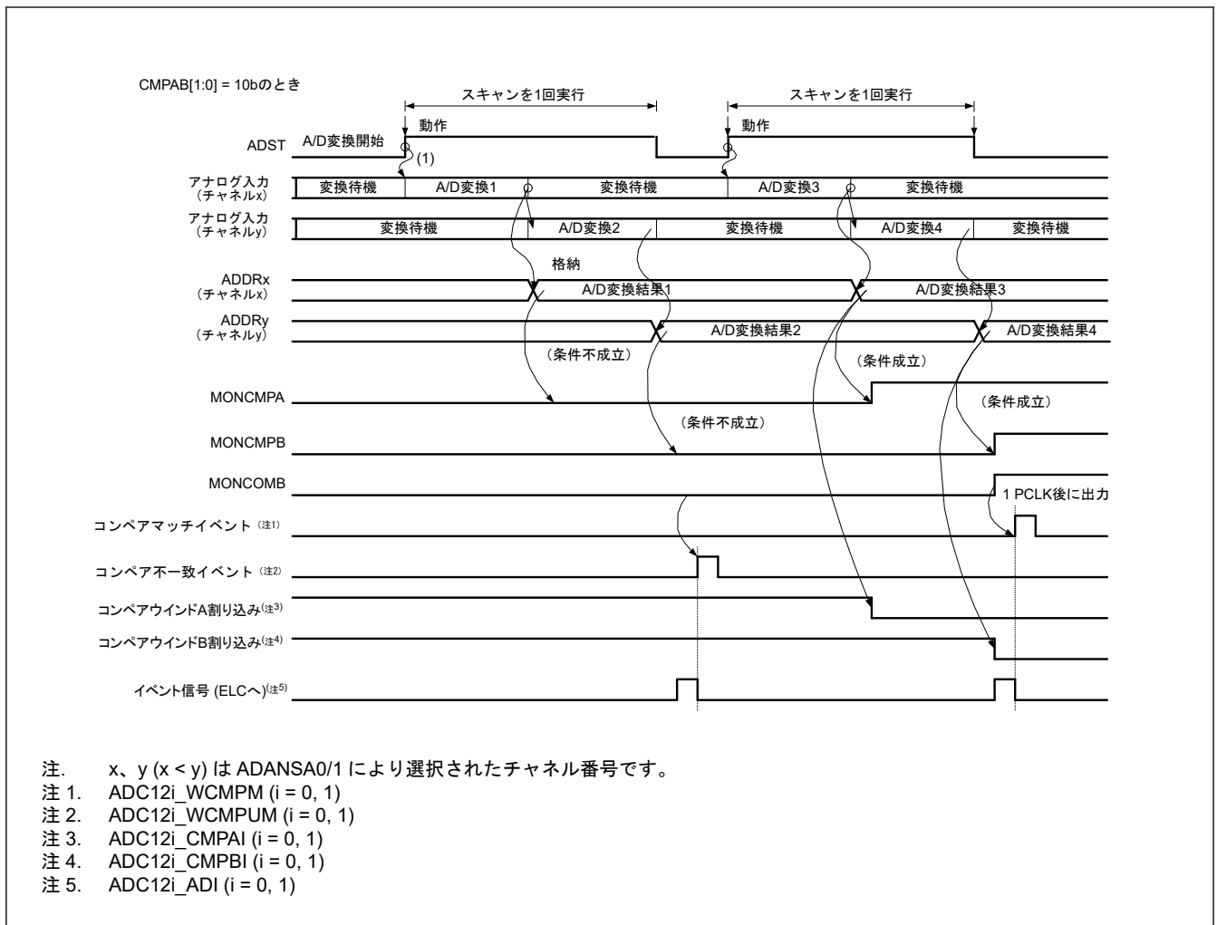
図 43.30 コンペア機能のイベント出力の動作例（アナログ入力（チャンネル x、y）を比較）
