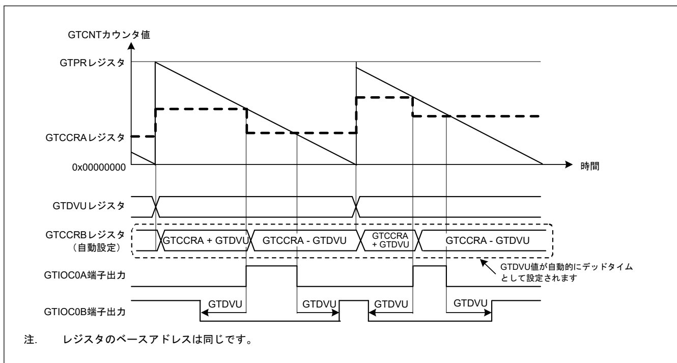
図 21.25 デッドタイム自動設定機能の動作例 (のこぎり波ワンショットパルスモード、ダウンカウント、アクティブ High の場合)
