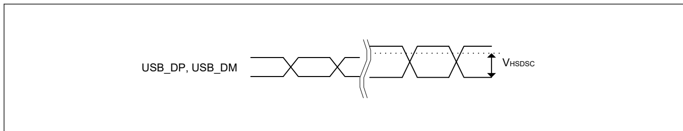
図 53.83 High-speed モードにおける USB_DP、USB_DM の切断検出感度
