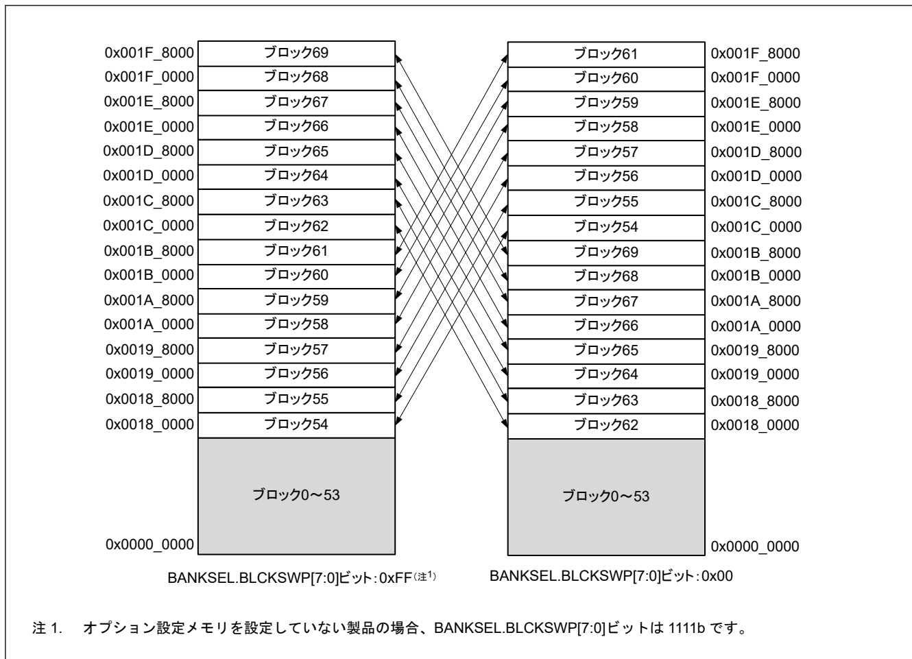
図 50.32 ブロックスワップ選択例 (2 M バイトのコードフラッシュメモリを持つ製品の場合)
