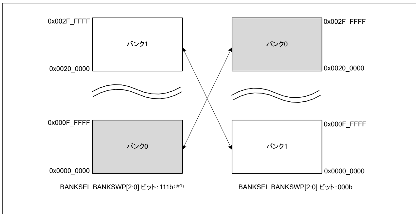
図 50.31 スタートアップバンク選択例 (2 M バイトのコードフラッシュメモリを持つ製品の場合)
