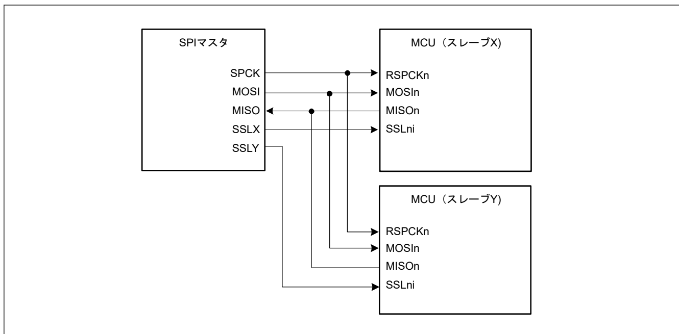
図 34.9 シングルマスタとマルチスレーブの構成例 (MCU はスレーブ)
