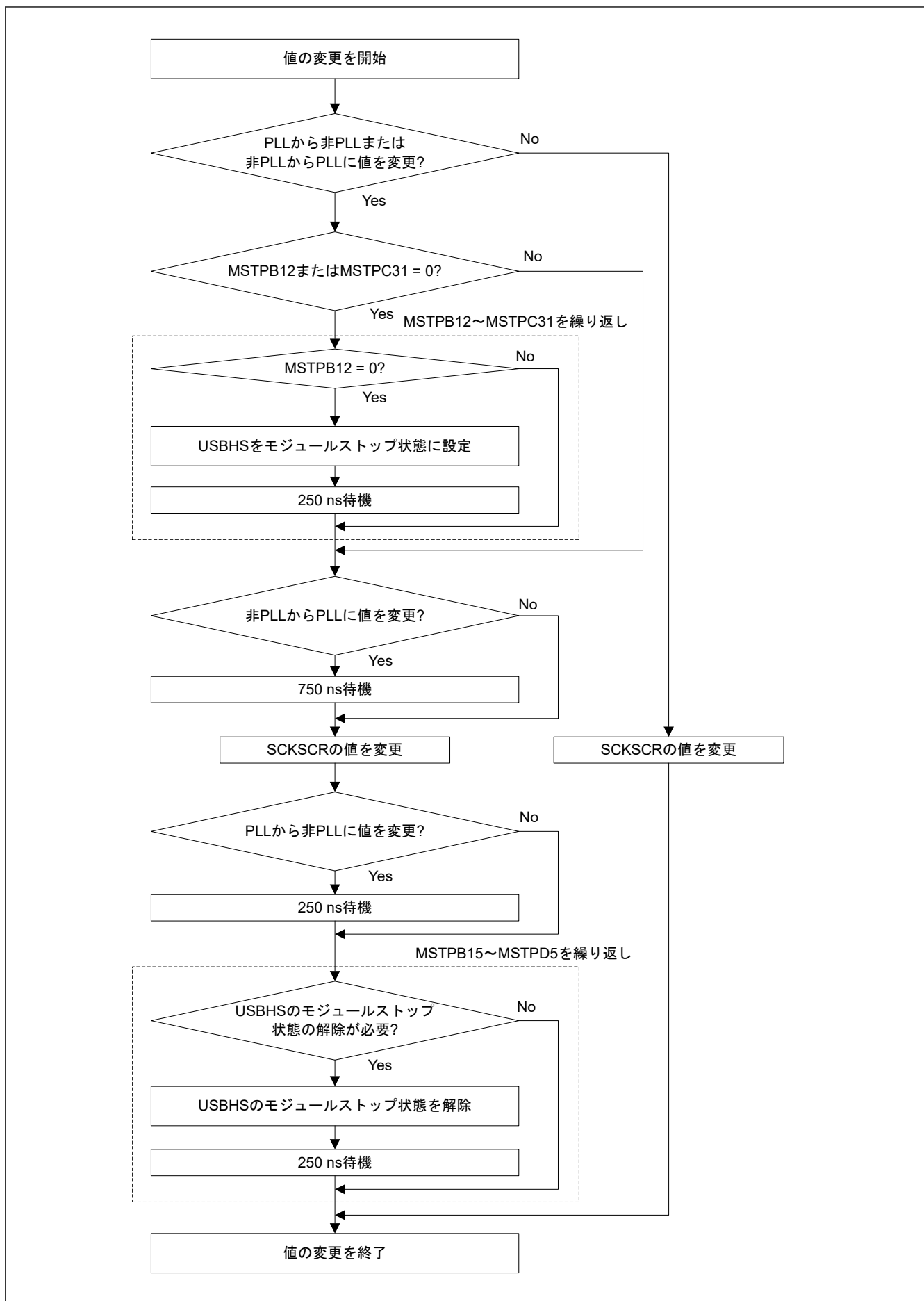
図 6.3 SCKSCRの値の変更フロー例
