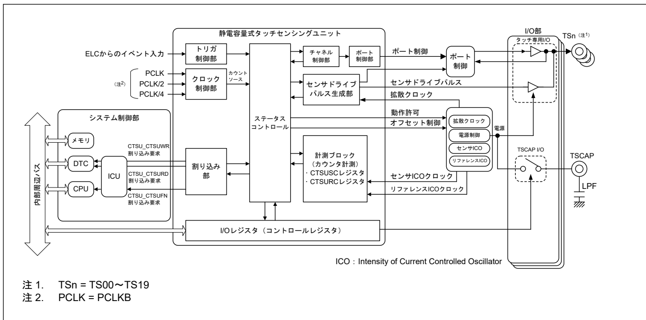
図 46.3 CTSU ブロック図
