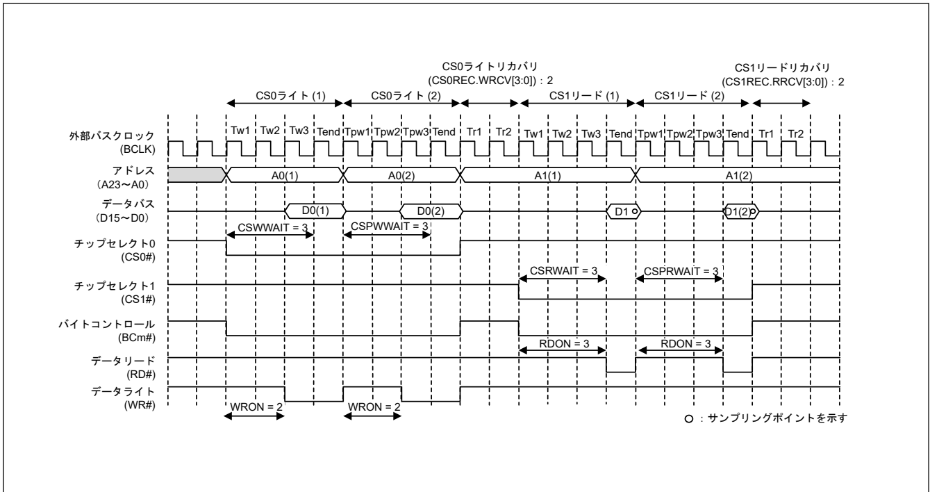
図 14.33 バスアクセスが分割された場合のリカバリサイクルの動作例（セパレートバスインタフェース、ページアクセスの場合）(m = 0~1)
