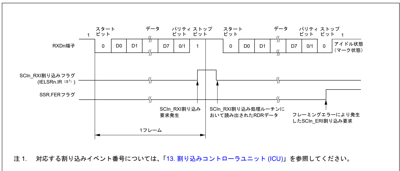
図 30.18 調歩同期式モードにおけるシリアル受信の動作例 (1) (RTS 機能を使用しない場合) (8 ビットデータ / パリティあり / 1 ストップビットの場合)
