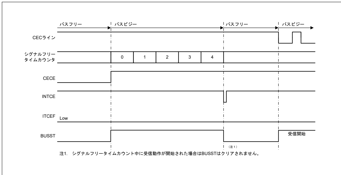
図 37.23 CECE = 1 時の受信開始時のタイミング
