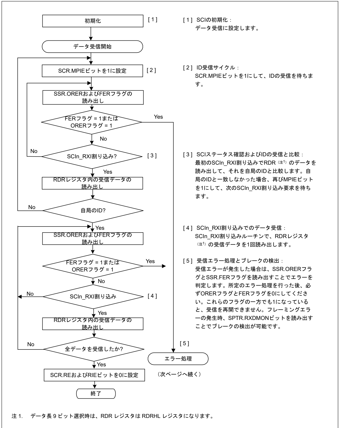
図 30.45 マルチプロセッサシリアル受信のフローチャート例 (非 FIFO 選択時) (1)
