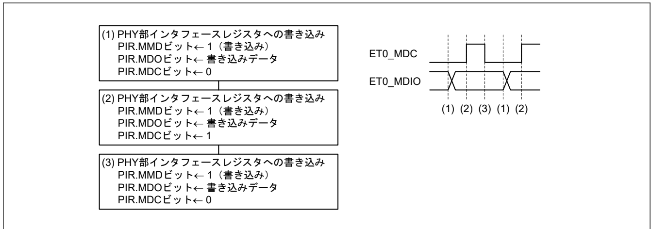
図 26.15 1 ビットデータの書き込みフロー
