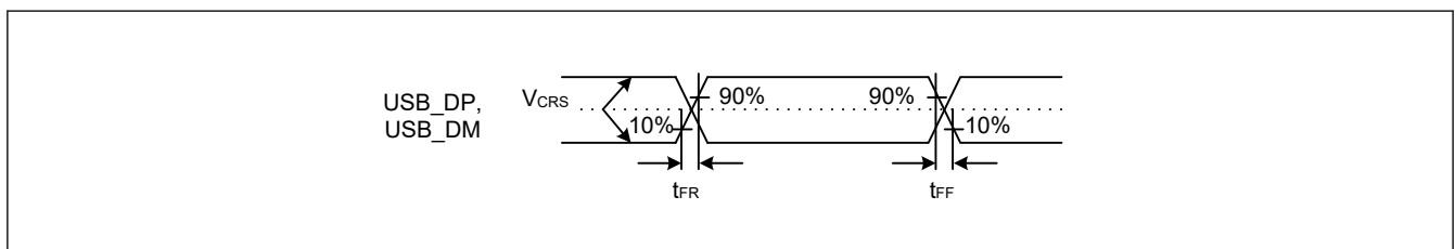
図 53.76 フルスピードモードにおける USB_DP、USB_DM の出力タイミング
