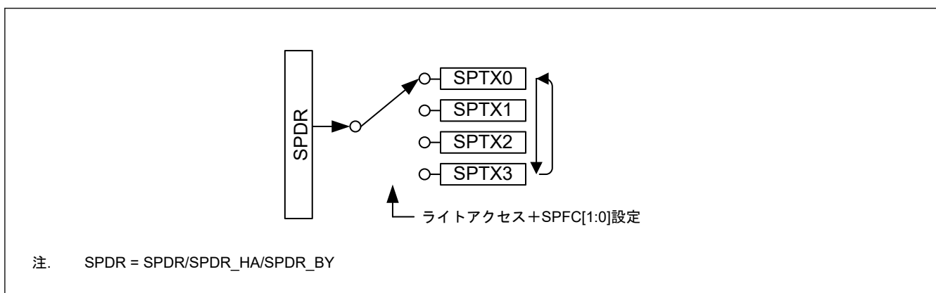
図 34.3 書き込み時の SPDR/SPDR_HA/SPDR_BY レジスタの構成図
