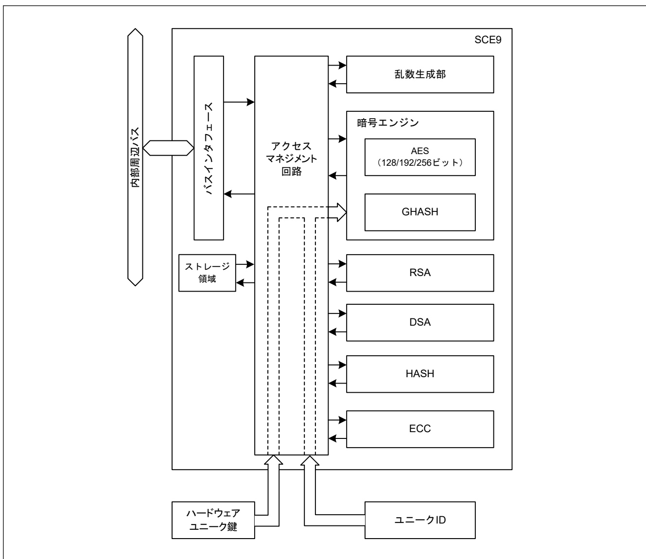
図 42.1 SCE9 のブロック図
