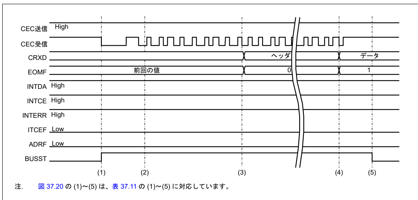
図 37.20 受信基本タイミング (2) (CECCTL0.CECRXEN = 1、ダイレクトアドレス、アドレス不一致、CECCTL1.CINTMK = 0)
