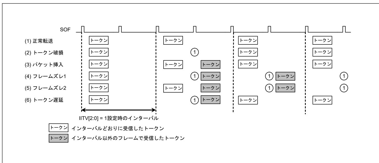
図 29.18 PIPEPERI.IITV[2:0] = 1 の場合のインターバルエラー発生例
