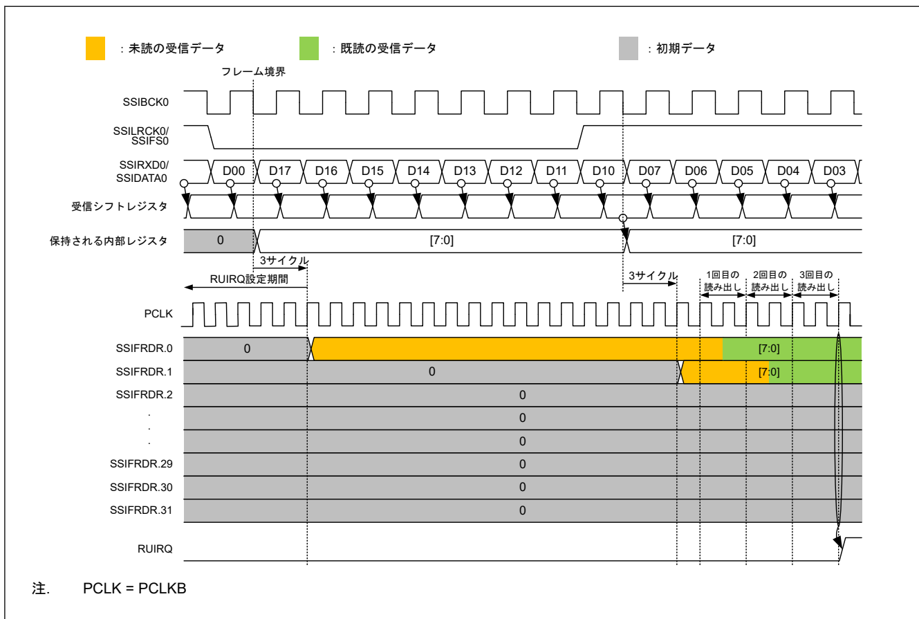
図 38.17 RUIRQ 設定タイミング
