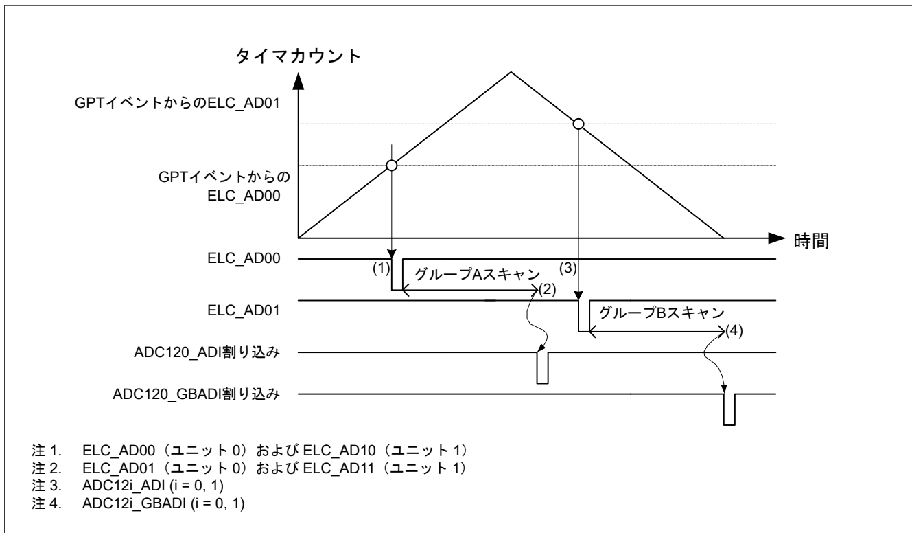
図 43.16 グループスキャンモードの基本動作例 (ELC からの同期トリガ使用)
