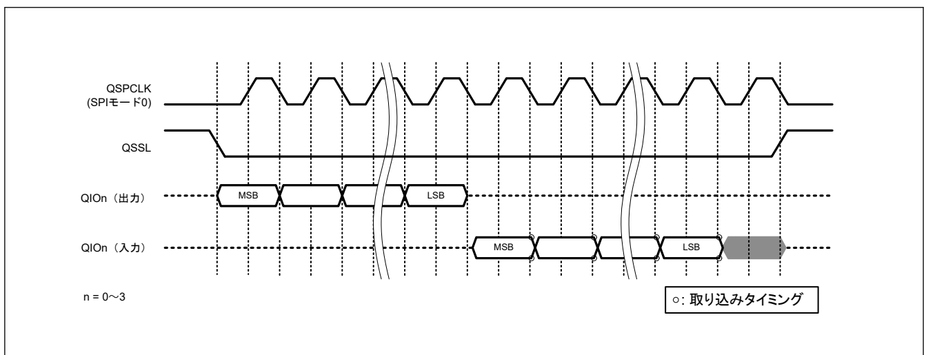
図 35.8 シリアルインタフェースの基本タイミング (SPI モード 0)
