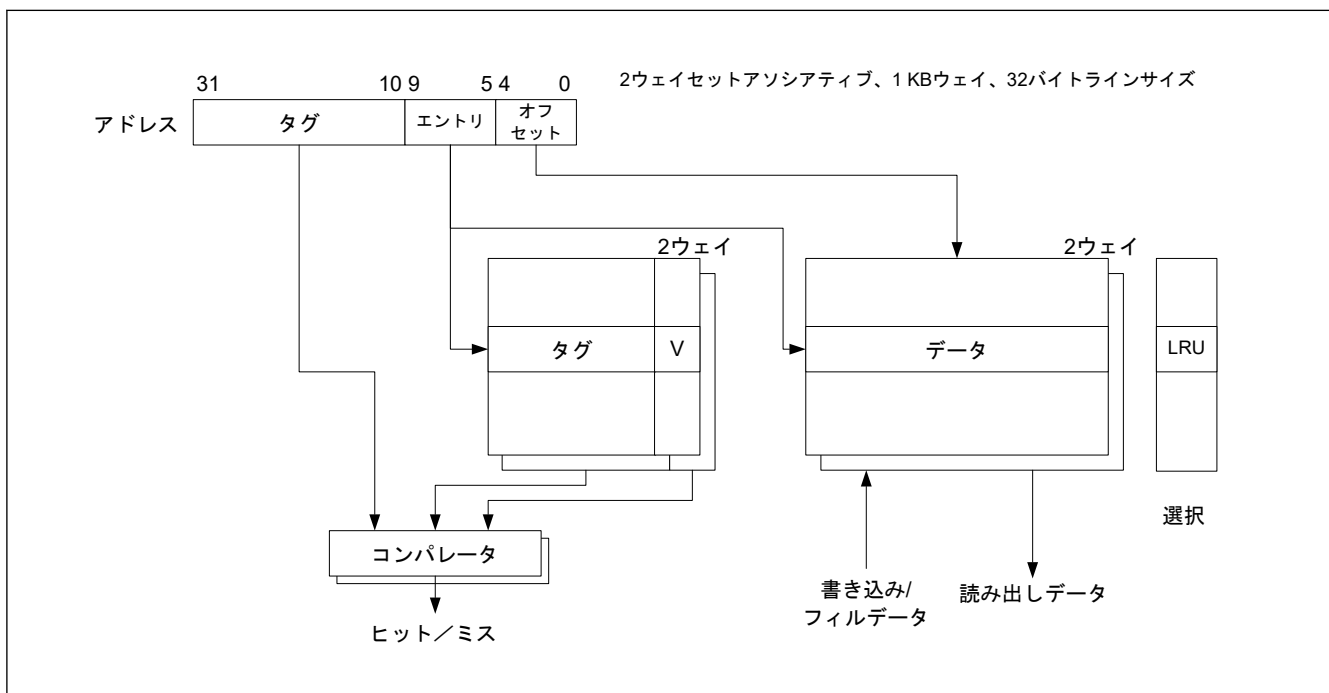
図 14.40 2 KB 容量、32 バイトラインサイズの 2 ウェイセットアソシアティブのキャッシュ構造
