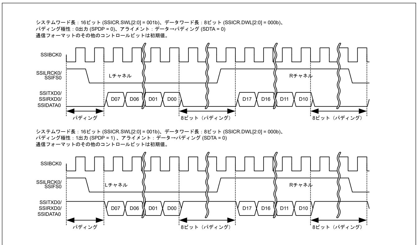
図 38.11 パディングビットの極性
