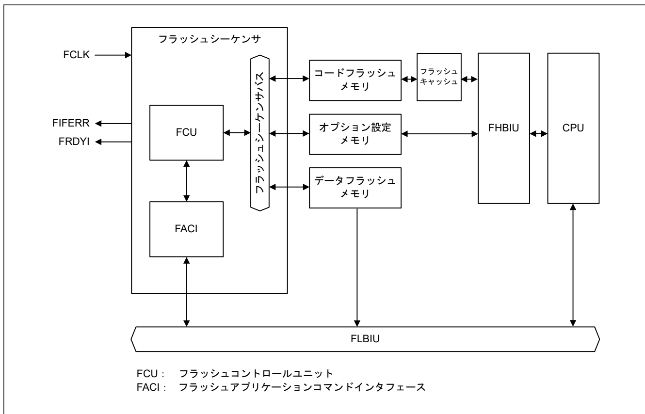
図 50.1 フラッシュメモリ関連モジュールのブロック図
