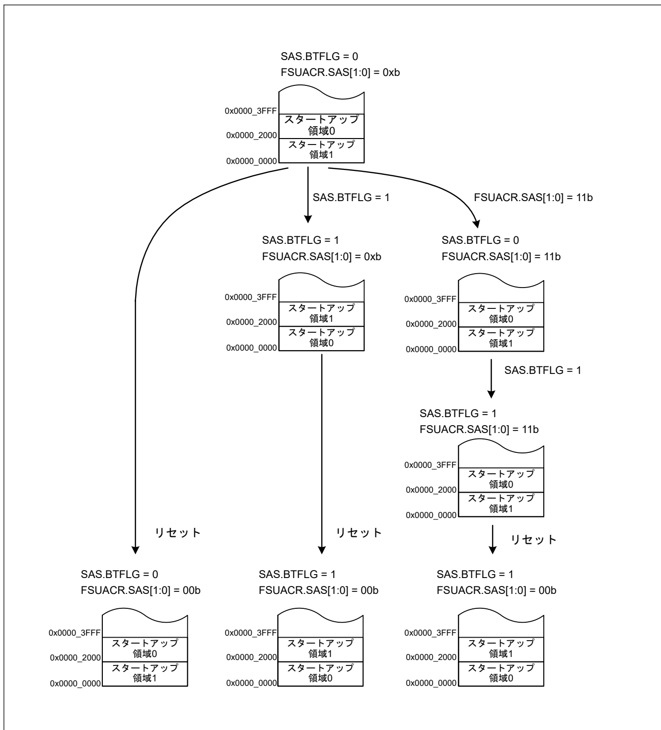
図 50.28 スタートアッププログラム保護設定の遷移例 2
