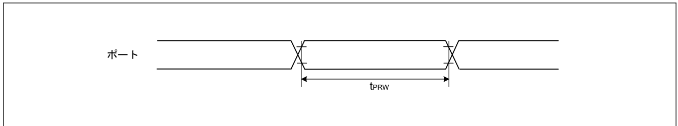
図 53.27 I/O ポート入力タイミング
