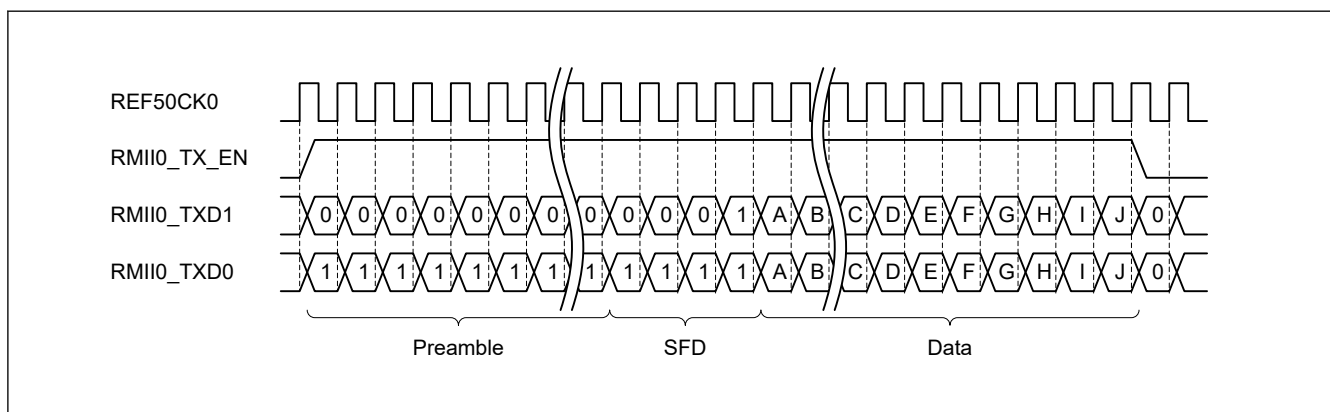
図 26.12 RMII フレーム送信タイミング (正常送信時)
