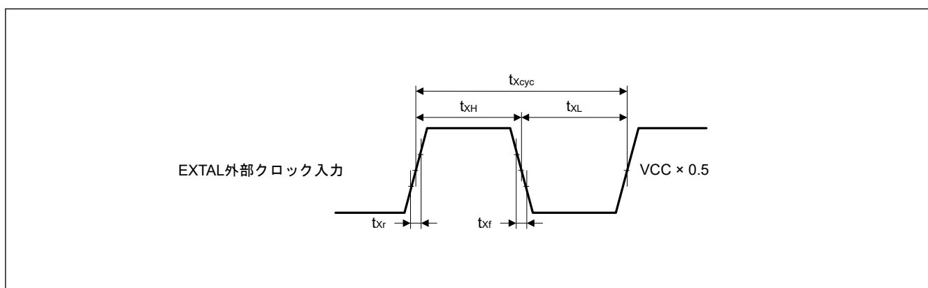
図 53.8 EXTERNAL 外部クロック入力タイミング
