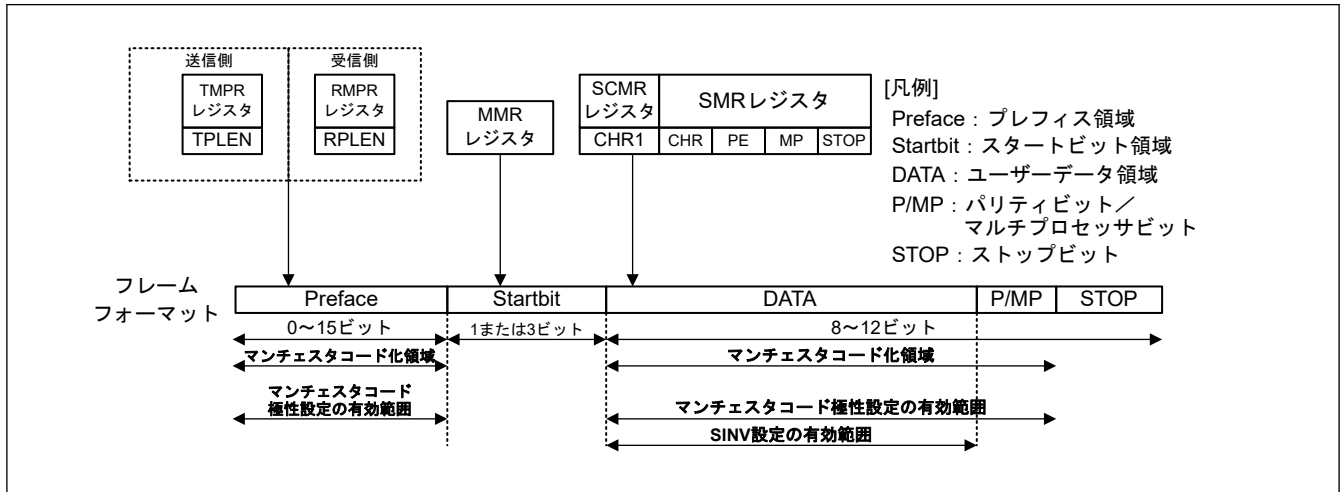
図 30.50 マンチェスタモードでのフレームフォーマット
