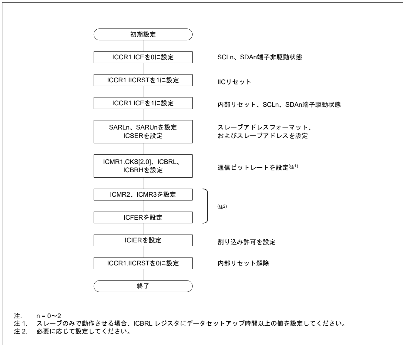
図 31.5 IIC の初期化フローチャート例
