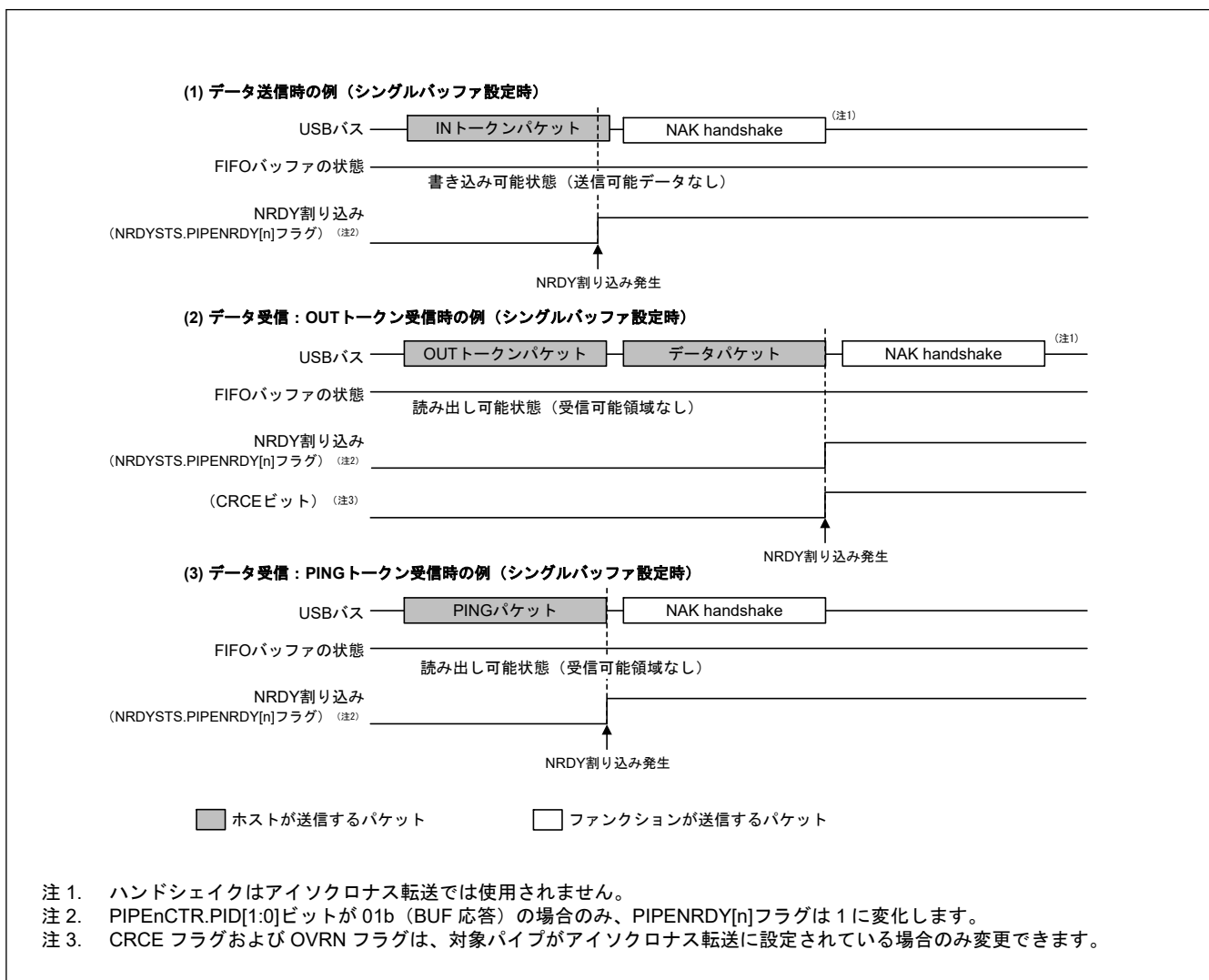
図 29.6 デバイスコントローラモード時の NRDY 割り込み発生タイミング
