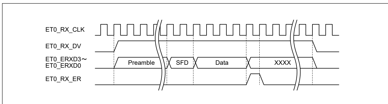
図 26.10 MII フレーム受信タイミング (受信エラー通知時)
