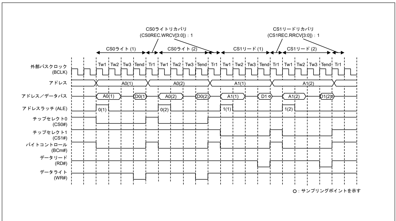
図 14.36 バスアクセスが分割された場合のリカバリサイクルの動作例（アドレス／データマルチプレクス I/O インタフェースの場合）(m = 0、1)
