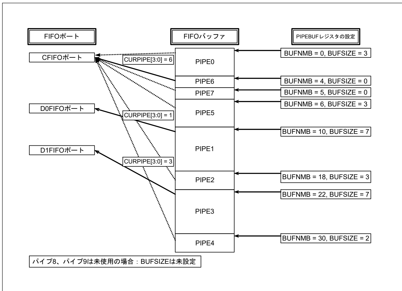
図 29.11 FIFO バッファのメモリマップ例
