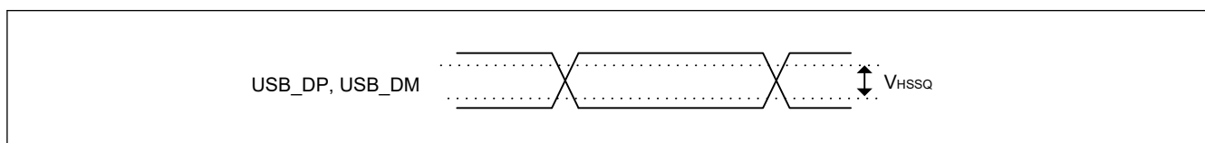
図 53.82 High-speed モードにおける USB_DP、USB_DM の Squelch 検出感度
