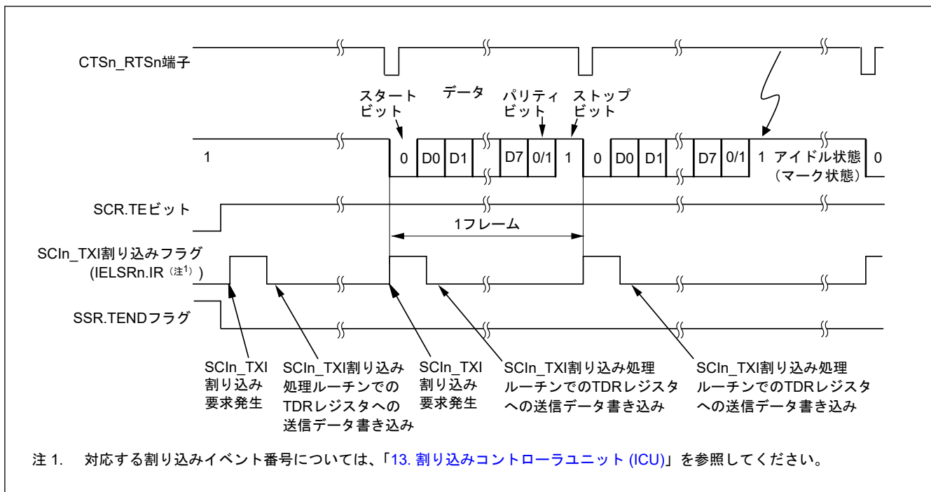
図 30.12 調歩同期式モードにおけるシリアル送信の動作例 (2) (8 ビットデータ/パリティあり/1ストップビット/CTS 機能使用/送信開始時)
