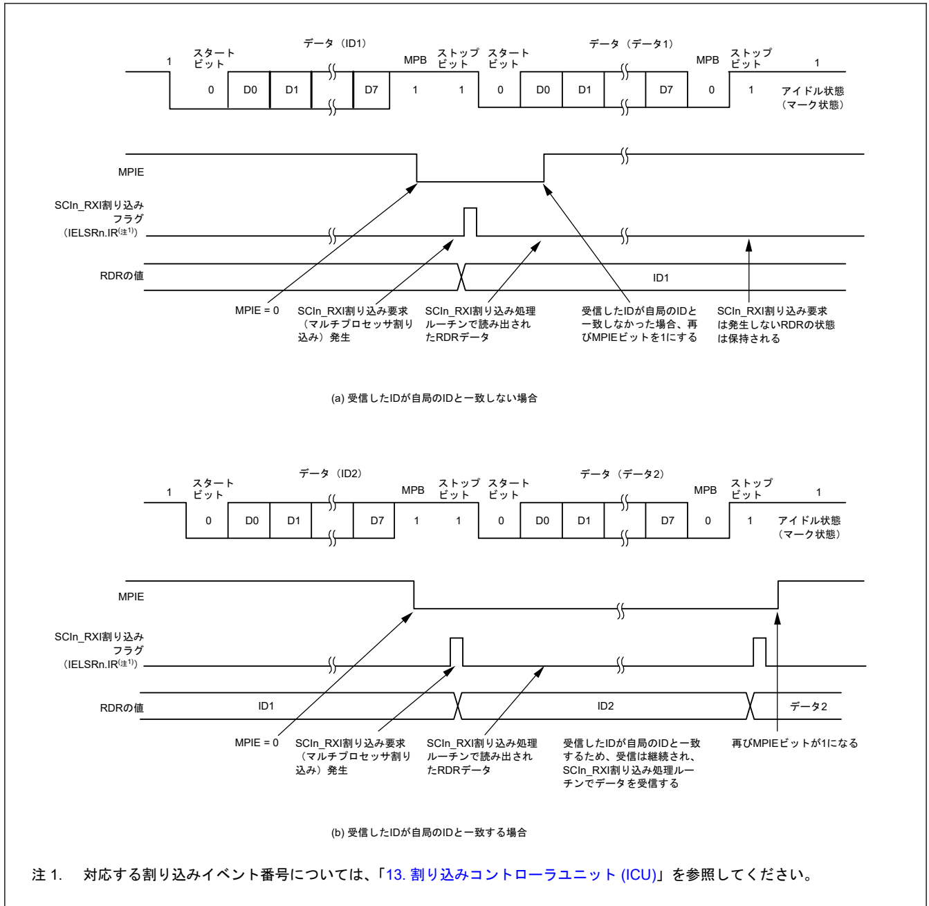
図 30.44 SCI の受信時の動作例 (8 ビットデータ/マルチプロセッサビットあり/1ストップビットの場合)
