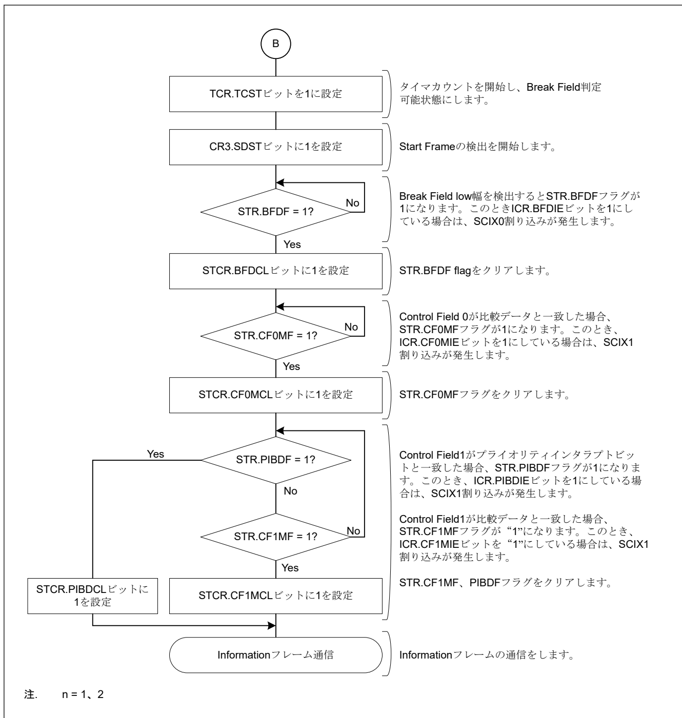
図 30.108 Start Frame 受信フローチャート例 (2)
