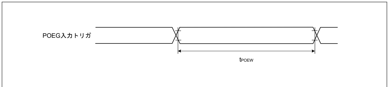
図 53.28 POEG 入力トリガタイミング
