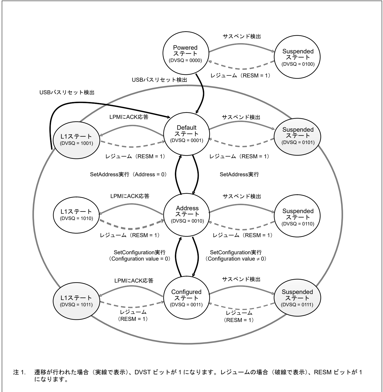
図 29.8 デバイスステートの遷移
