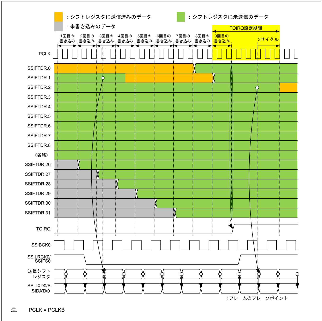
図 38.18 TOIRQ 設定タイミング
