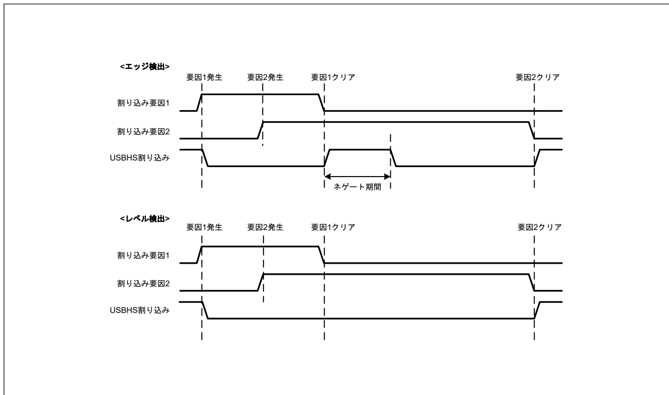
図 29.3 USBHS 割り込み動作
