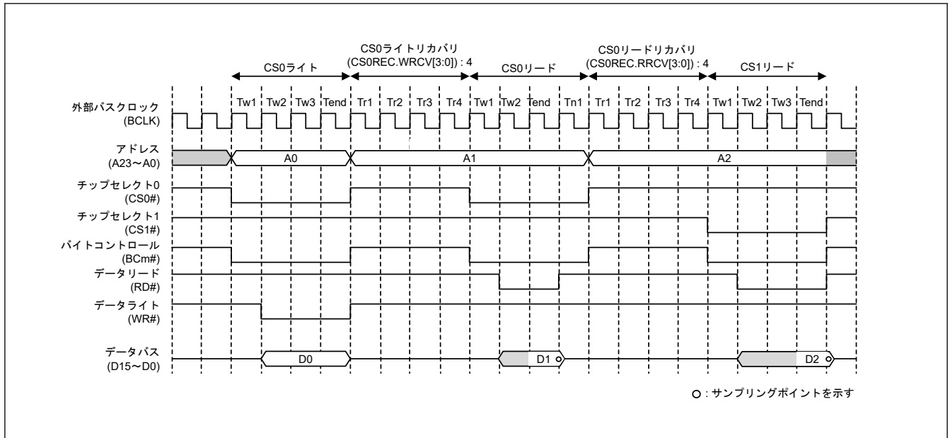
図 14.31 セパレートバスインタフェース時のリカバリサイクルの動作例 (m = 0~1)
