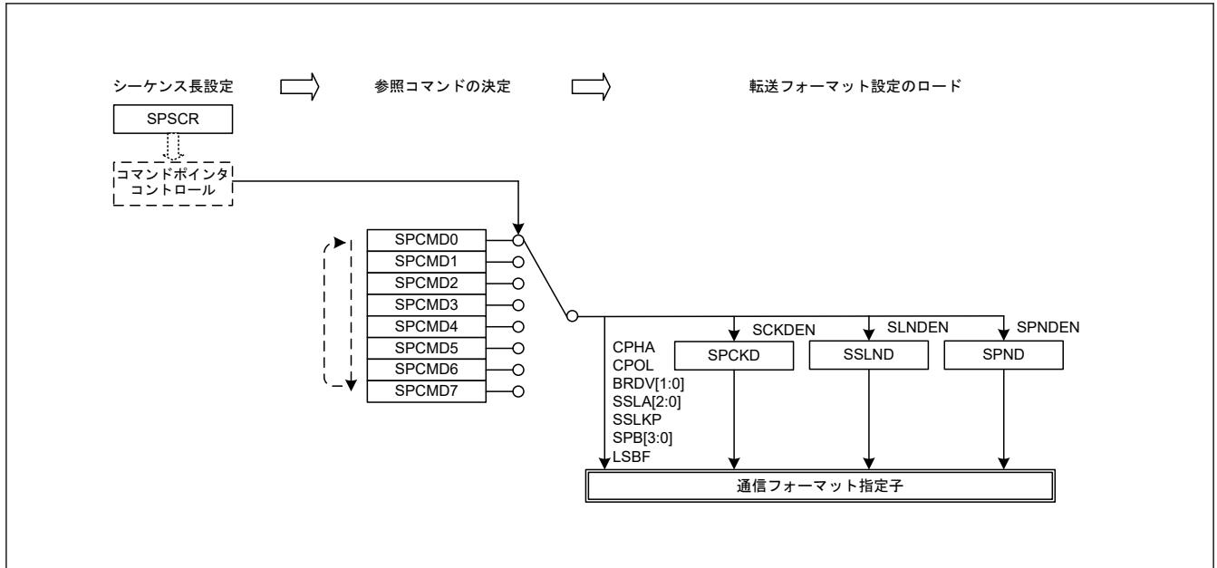
図 34.43 マスタモードでのシリアル転送方式の決定方法
