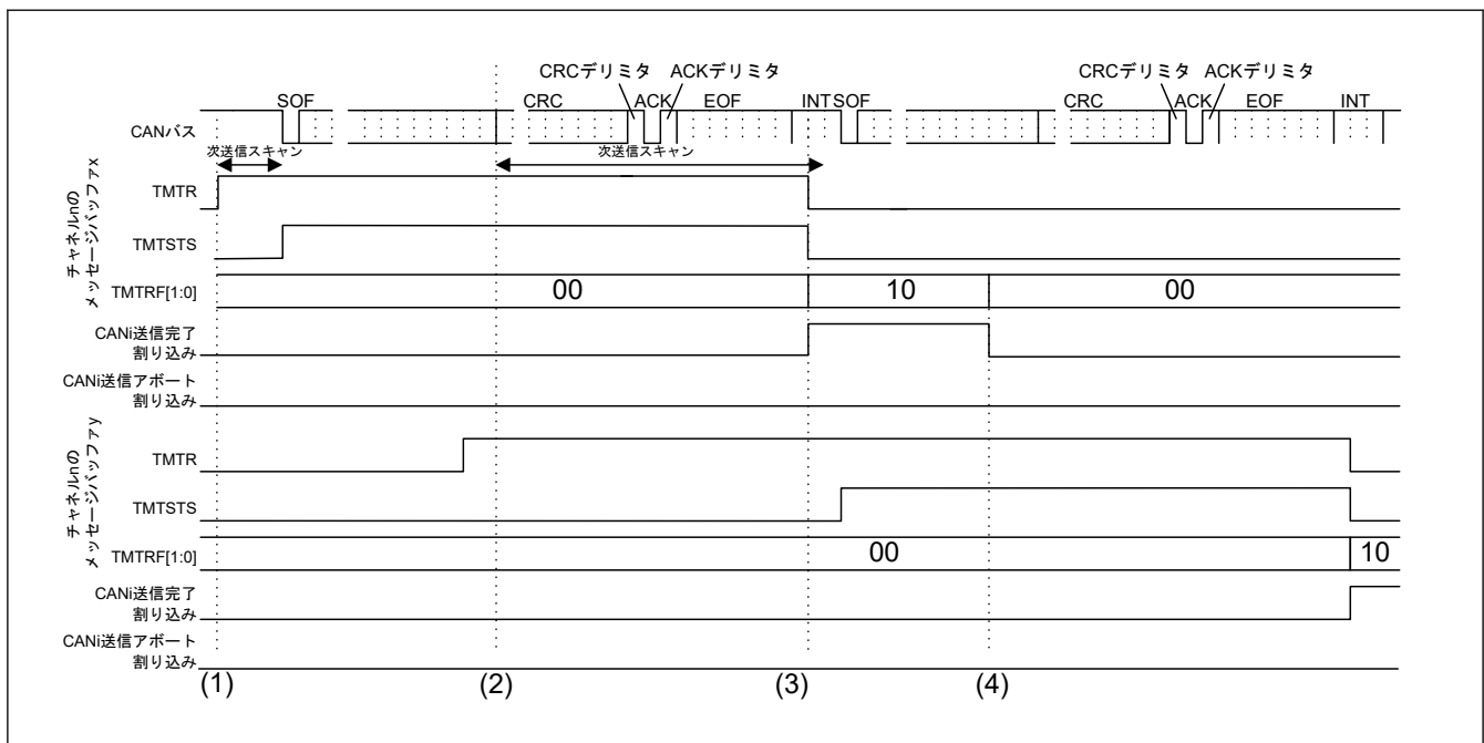
図 32.42 正常送信の要求およびフラグビットのタイミング
