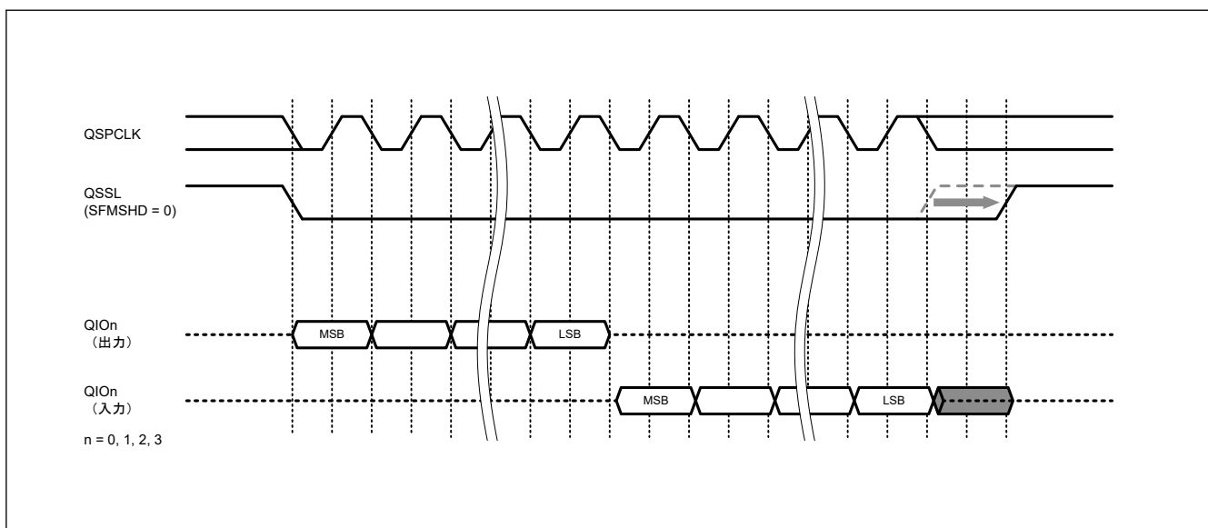
図 35.12 SFMSHD ビットを使用した QSSL 信号のホールド時間調整
