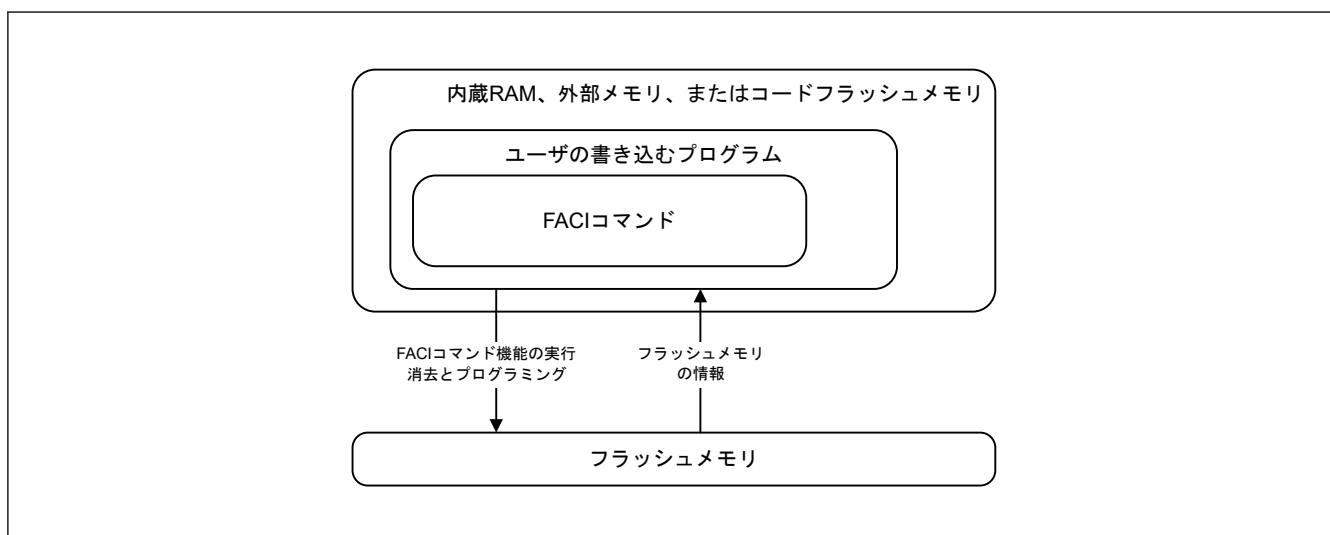
図 50.46 セルフプログラミングの概念
