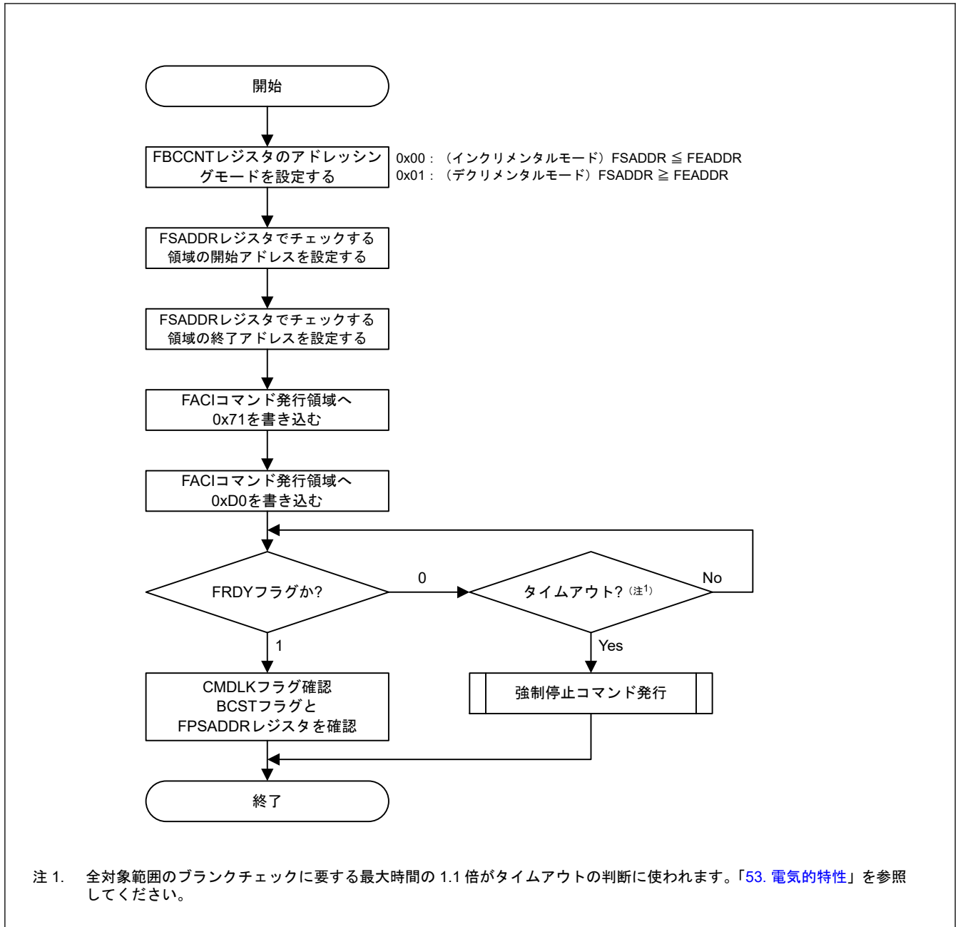
図 50.24 ブランクチェックコマンドの使用フロー
