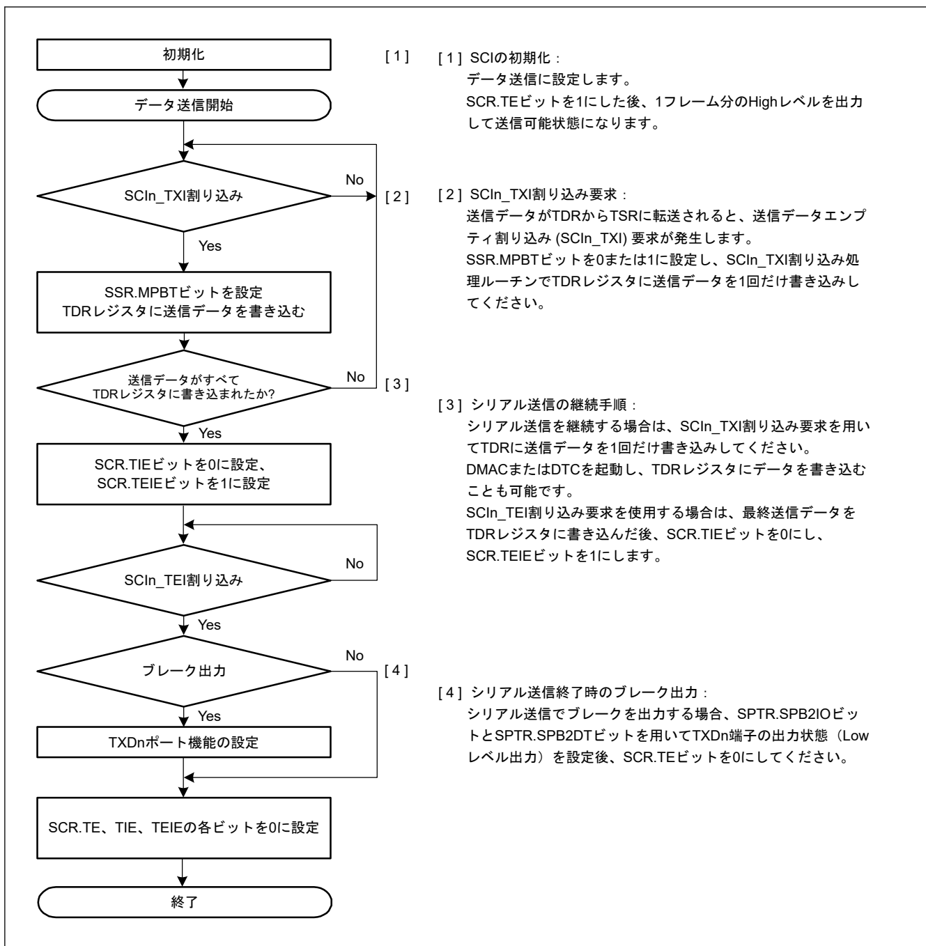
図 30.41 マルチプロセッサシリアル送信のフローチャート例 (非 FIFO 選択時)
