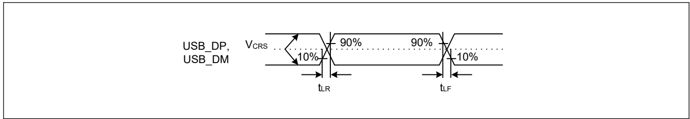
図 53.74 Low-speed モードにおける USB_DP、USB_DM の出力タイミング
