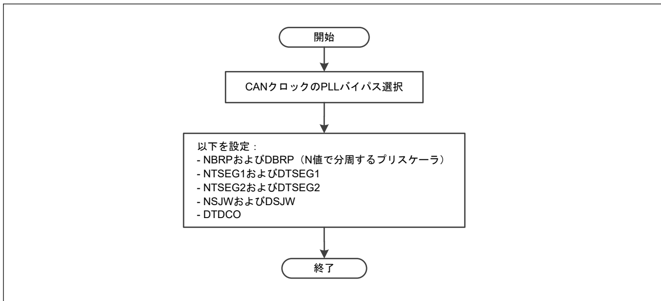
図 32.17 CAN のビットタイミングとボーレートを設定する手順
