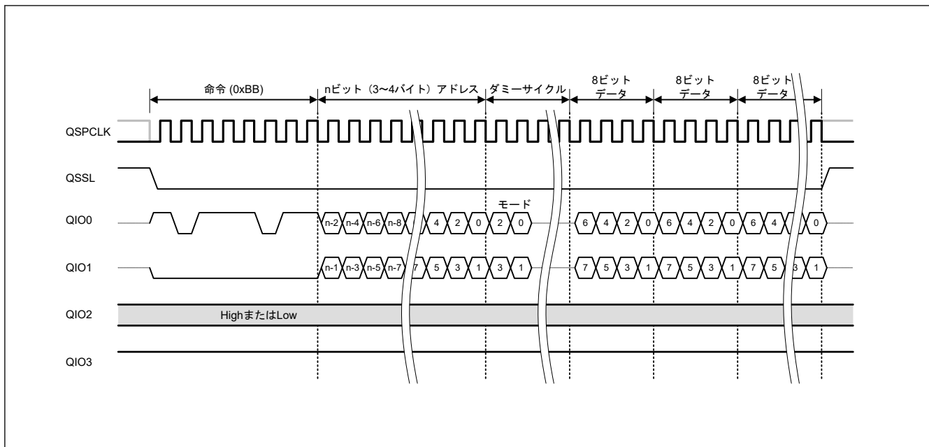
図 35.23 ファストリード Dual I/O バスサイクル(拡張 SPI プロトコル時)
