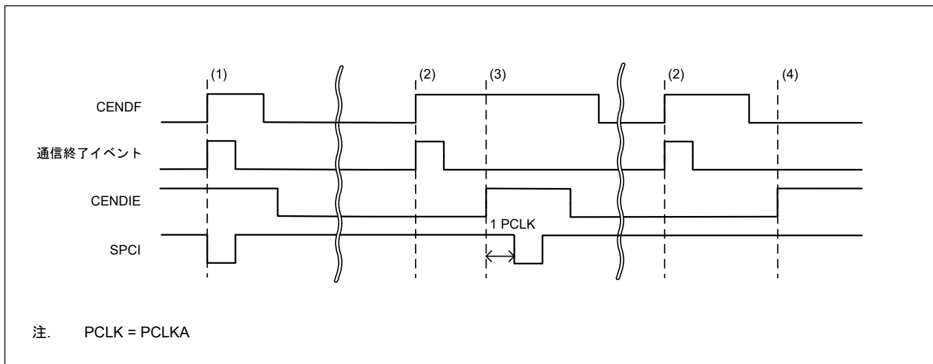
図 34.36 通信終了割り込みの動作例 (イネーブル制御)
