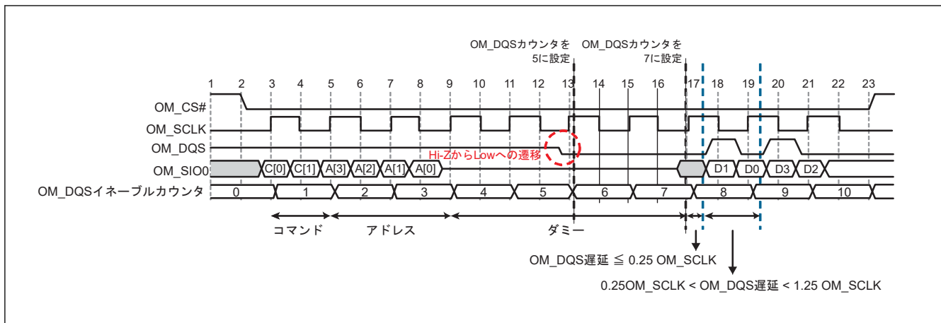
図 36.22 OM_DQS クロック入力が Hi-Z から Low に遷移するタイミングの例 (フラッシュ DOPI モード、ダミーサイクル数 = 4、OM_DQS プレサイクル ON)
