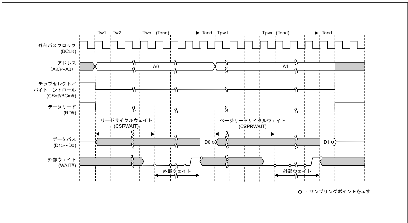
図 14.26 16 ビットバス空間に対するページリードアクセスの外部ウェイトタイミング例 (EBCLK 端子出力選択ビットで BCLK の 1 分周を選択した場合) (n = 0~7, m = 0, 1)
