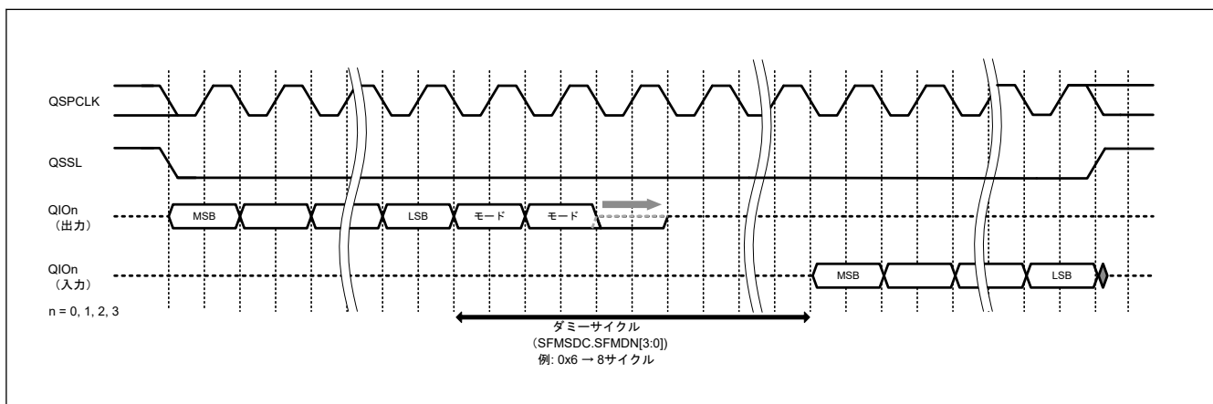
図 35.14 SFMOEX ビットを使用した出力許可ホールド時間調整 (ファストリード)
