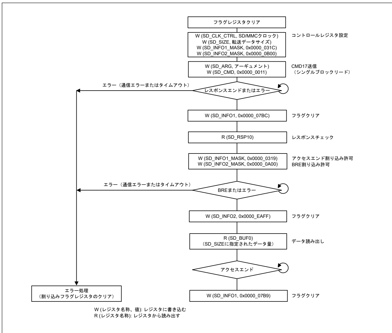
図 39.11 シングルブロックリード動作のフロー例
