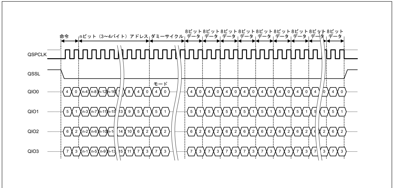
図 35.7 Quad-SPI プロトコル例 (ファストリード Quad I/O)
