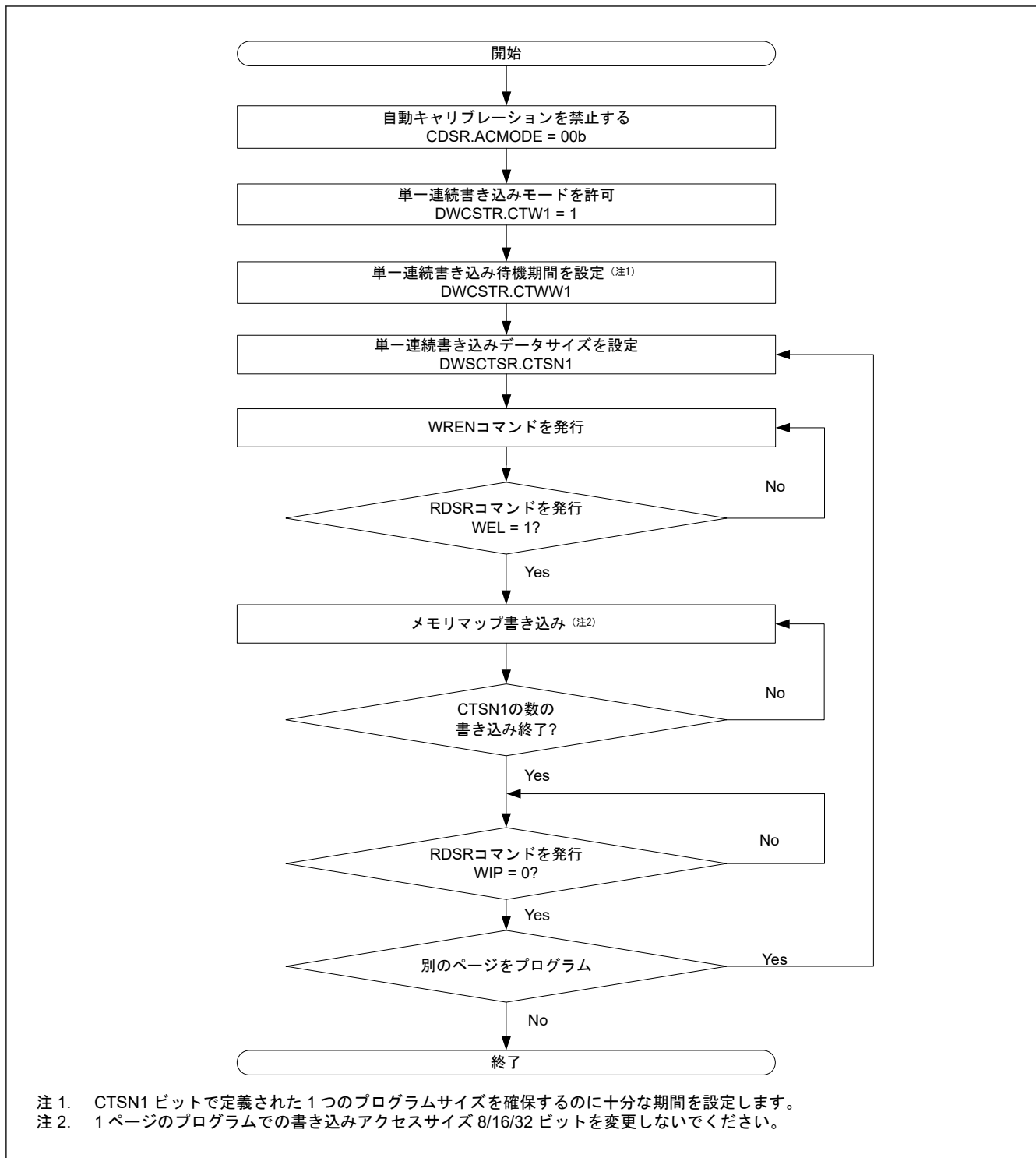
図 36.17 OctaFlash プログラムの手順
