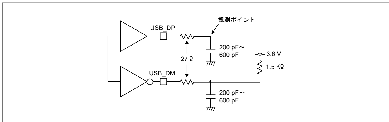
図 53.79 Low-speed モードにおける測定回路
