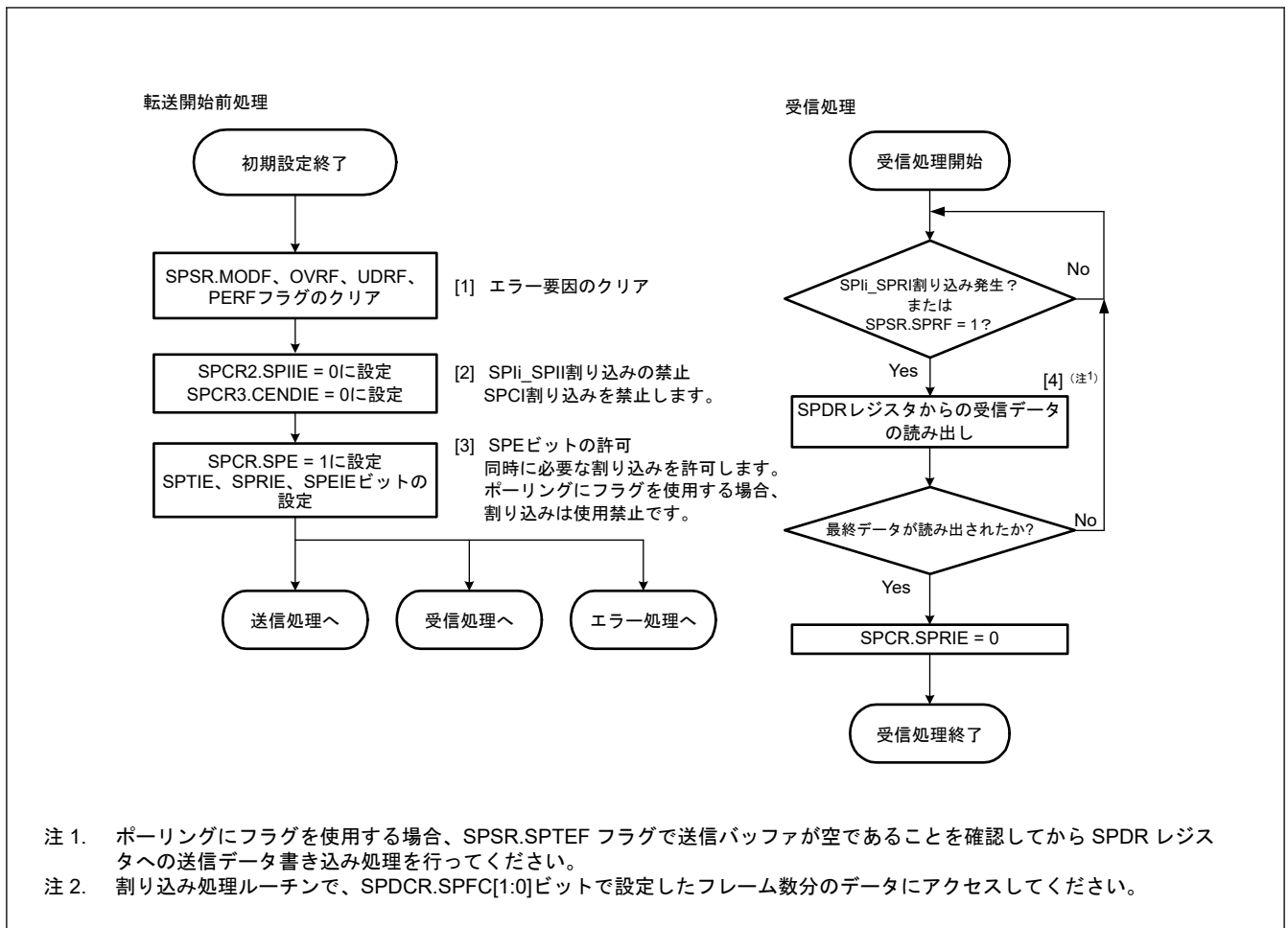
図 34.54 スレーブモードでの受信フロー
