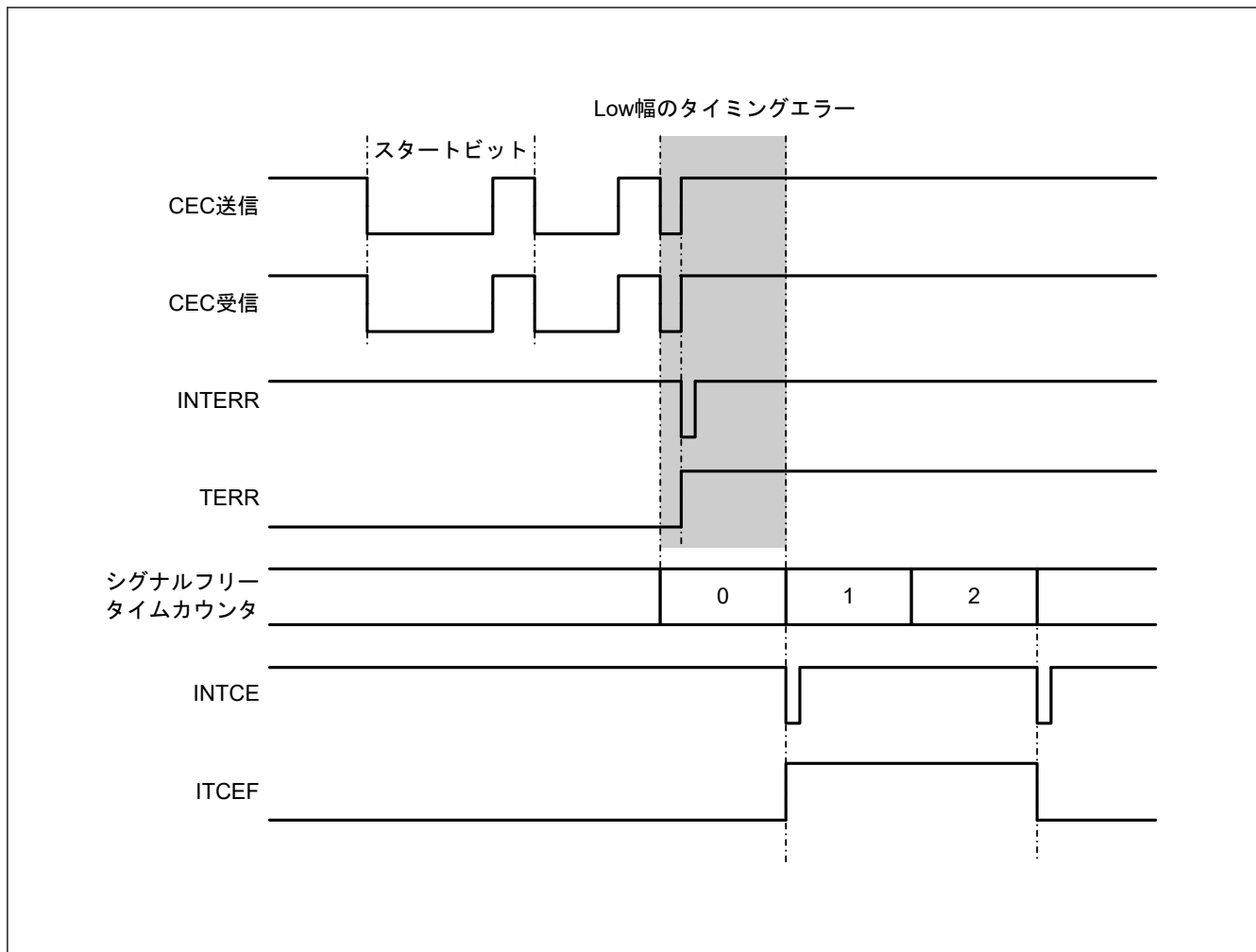
図 37.40 イニシエータ動作時のタイミングエラー
