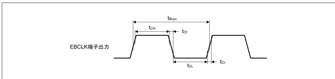
図 53.7 EBCLK 出力タイミング
