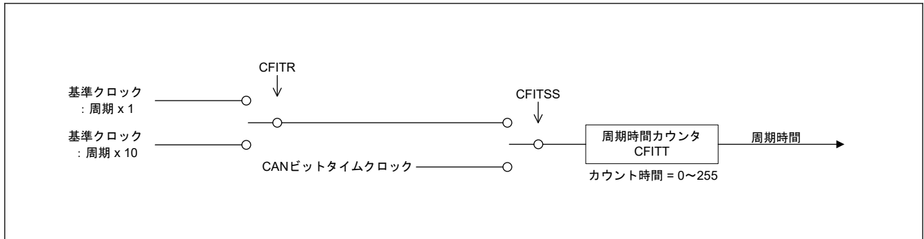
図 32.46 FIFO インターパルタイマのブロック図
