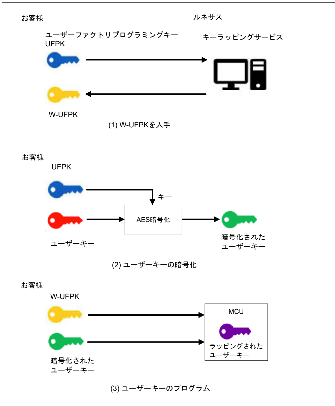
図 52.3 キーインジェクション
