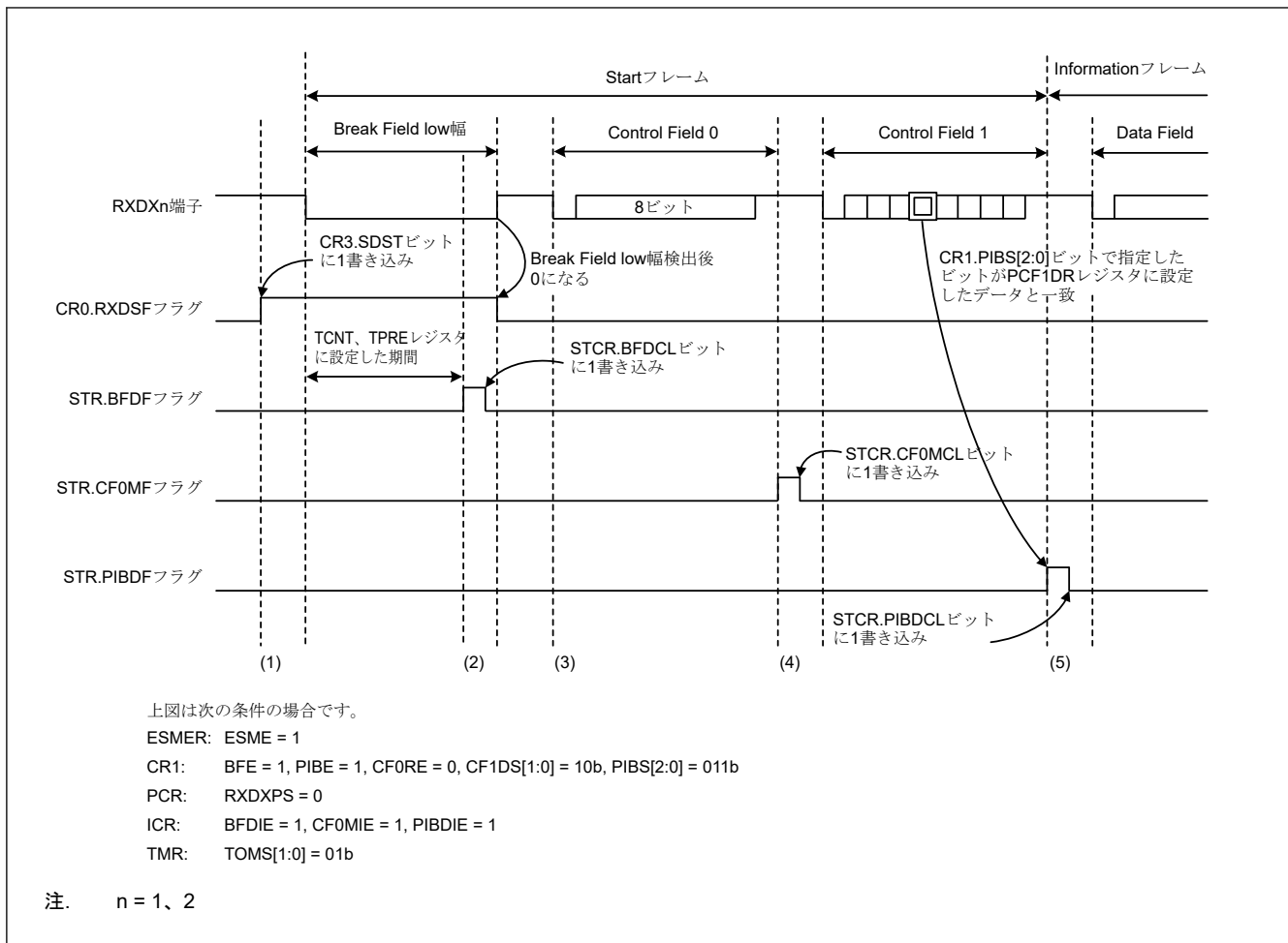
図 30.110 Start Frame の受信時の動作例（プライオリティインタラプトビット使用時）
