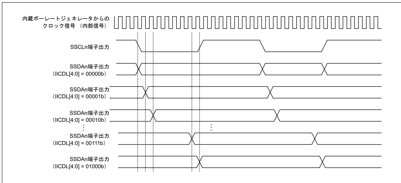
図 30.92 SDA n 出力遅延のタイミング
