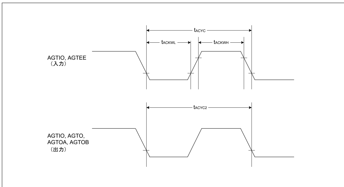
図 53.32 AGT 入出力タイミング
