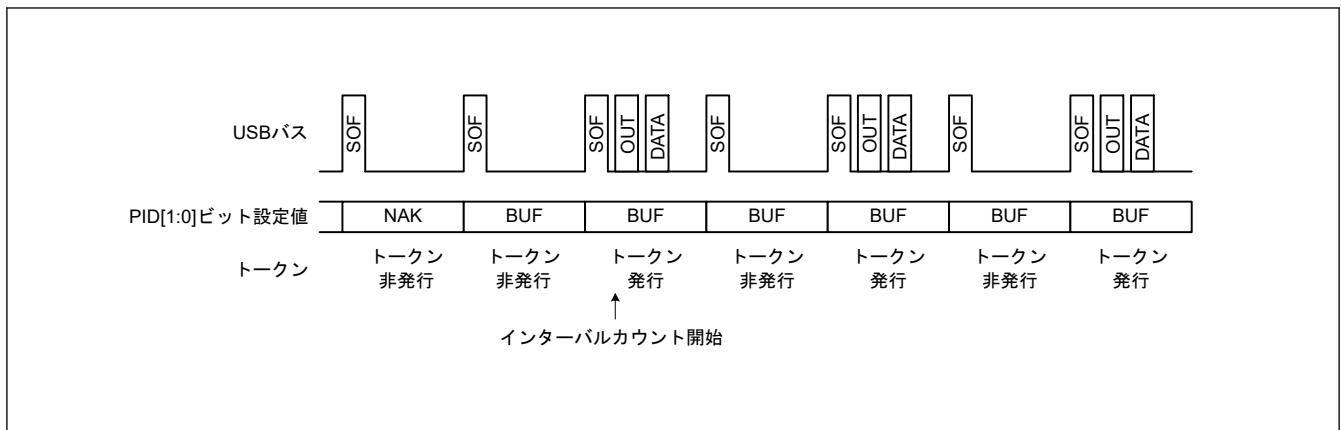
図 29.13 IITV[2:0] = 1 の場合におけるトークン発行の有無
