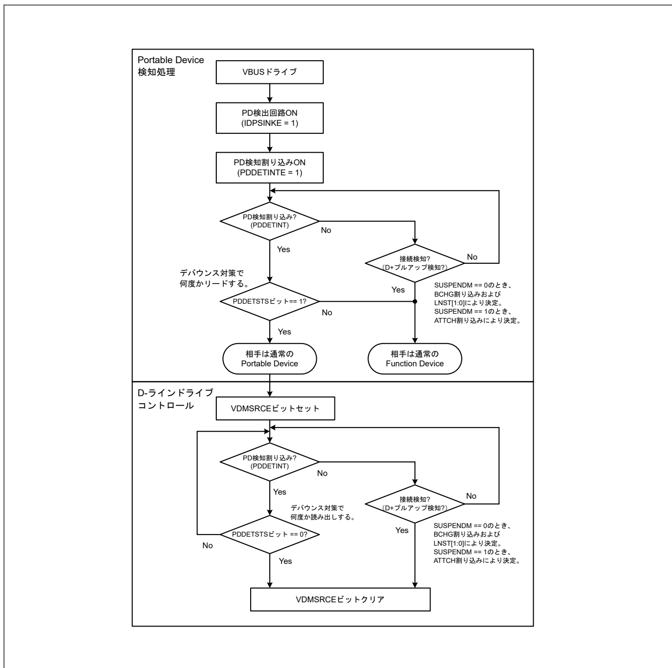
図 29.21 ハードウェアに Portable Device 検出機能搭載時の Charging Downstream ポート処理フロー
