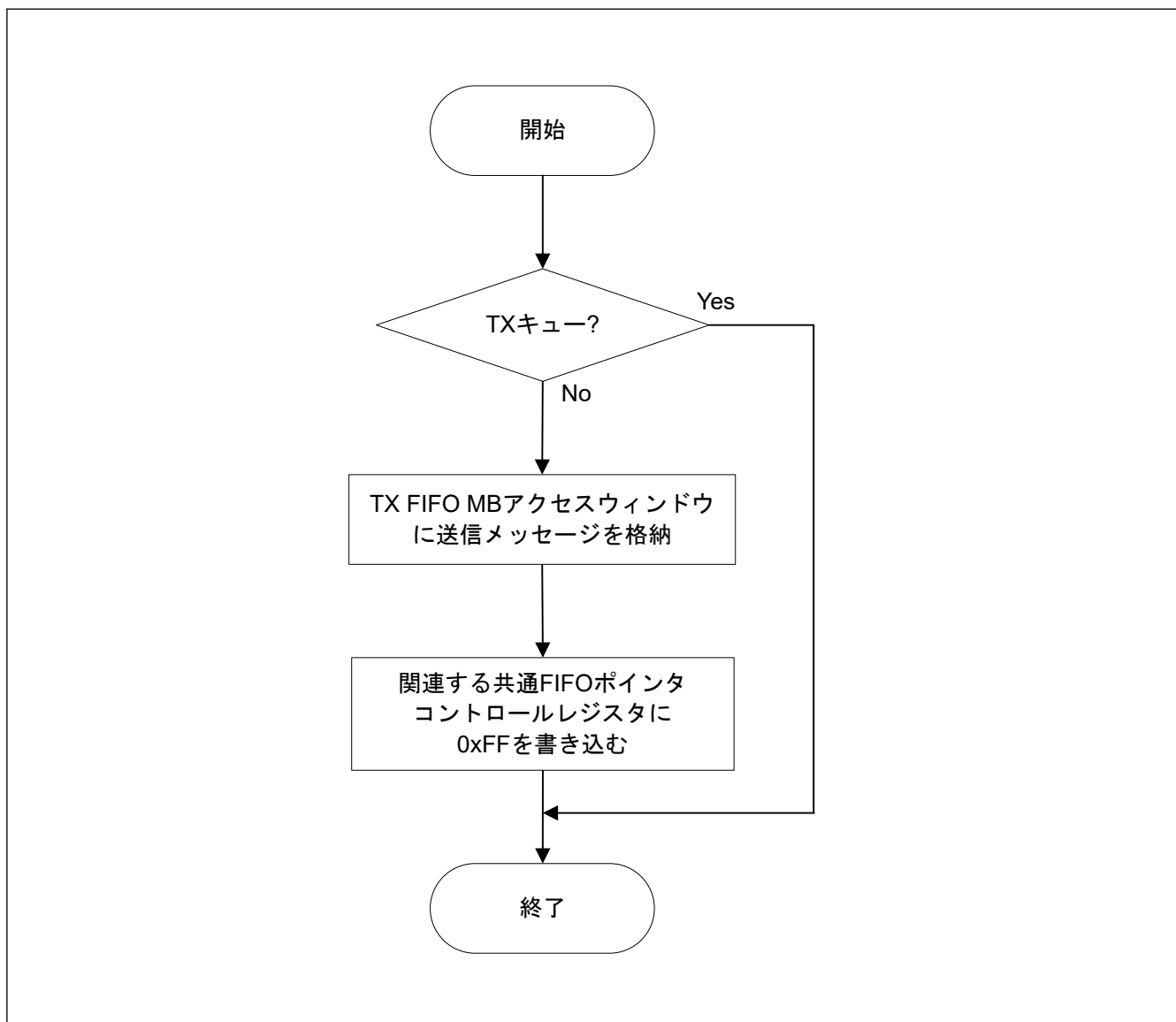
図 32.44 TX FIFO の送信要求手順
