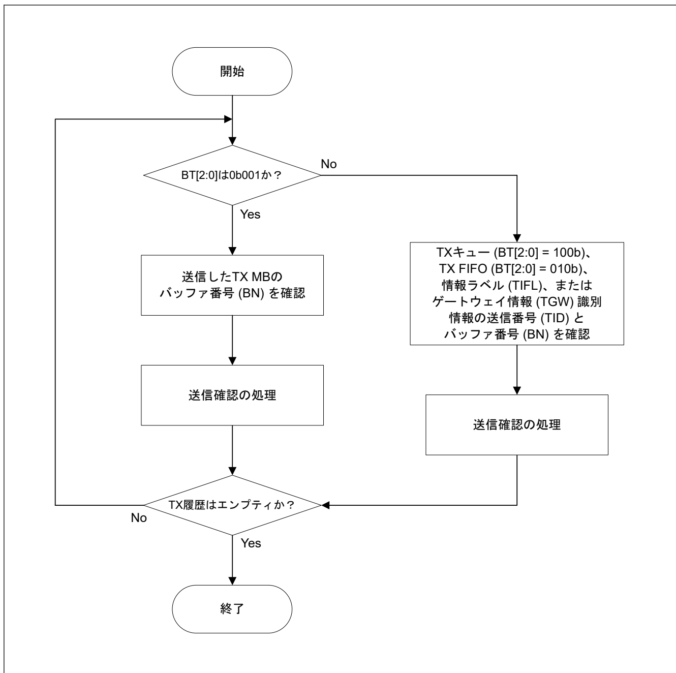
図 32.49 TX 履歴リストの処理手順
