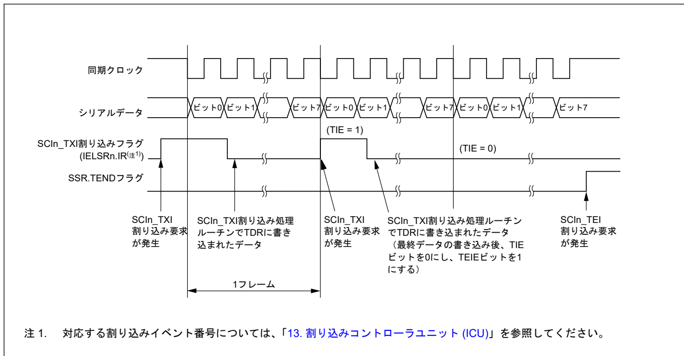
図 30.68 クロック同期式モードにおけるシリアル送信の動作例 (送信中～送信終了時)
