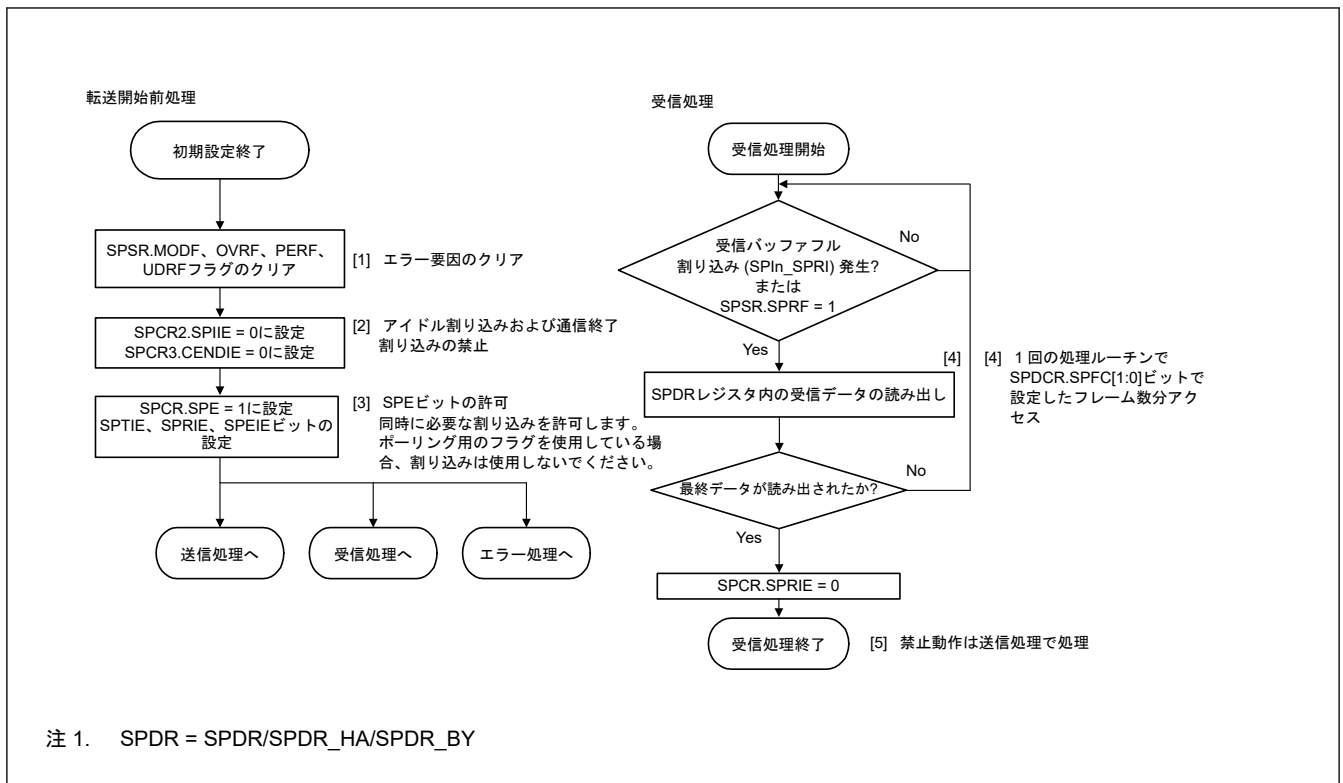
図 34.50 マスタモードでの受信フロー
