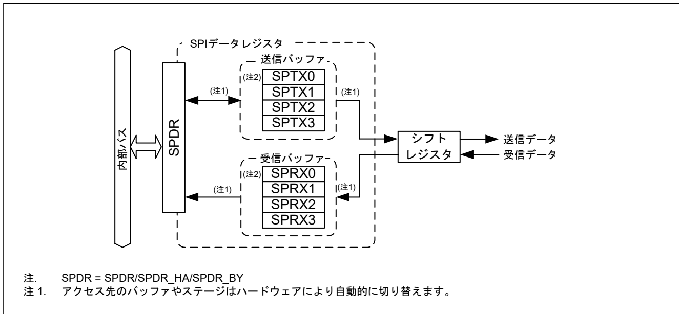
図 34.2 SPDR/SPDR_HA/SPDR_BY レジスタの構成図
