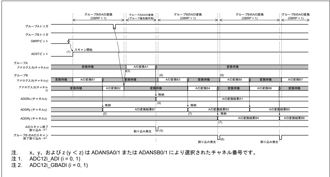
図 43.23 グループ優先動作の例 1-5 : グループ B のシングルスキャン連続動作 (ADGSPCR.GBRP = 1、ADGSPCR.LGRRS = 0 の場合)
