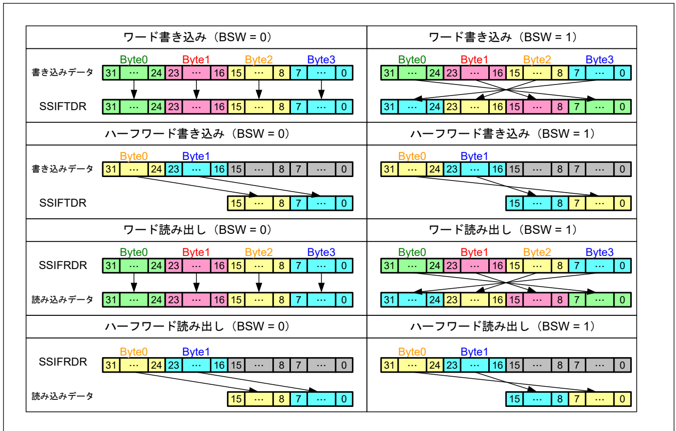
図 38.24 バイトスワップの動作例
