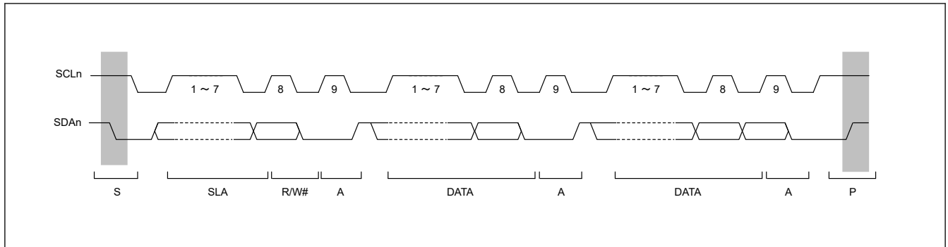
図 31.4 I 2 C バスタイミング (SLA = 7 ビットの場合)
