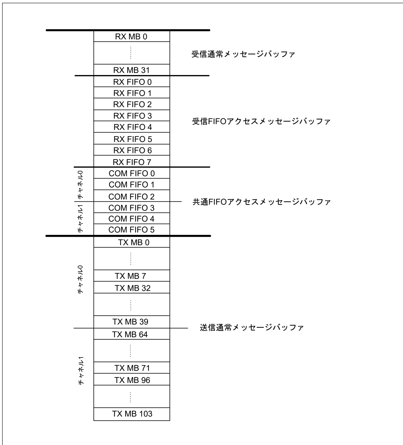
図 32.28 メッセージバッファの構成
