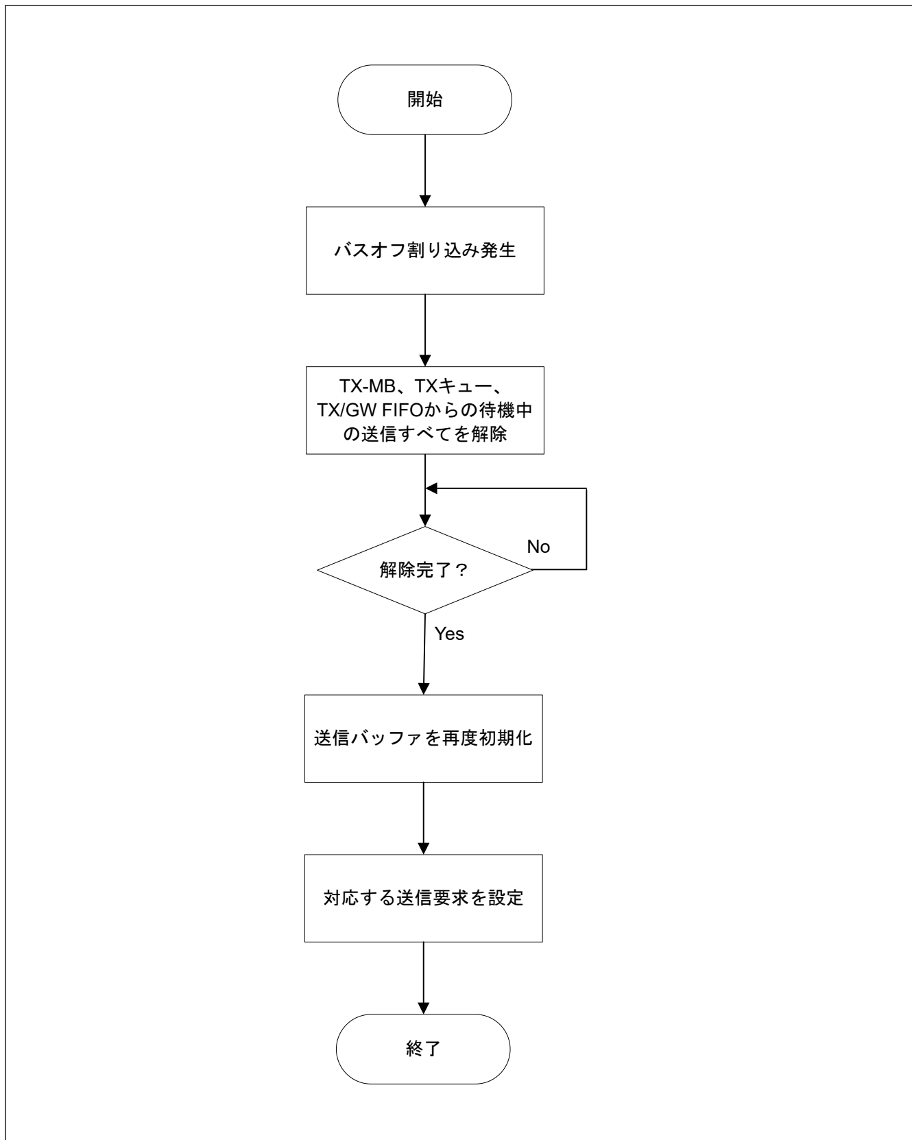
図 32.13 バスオフ中の送信の再初期化
