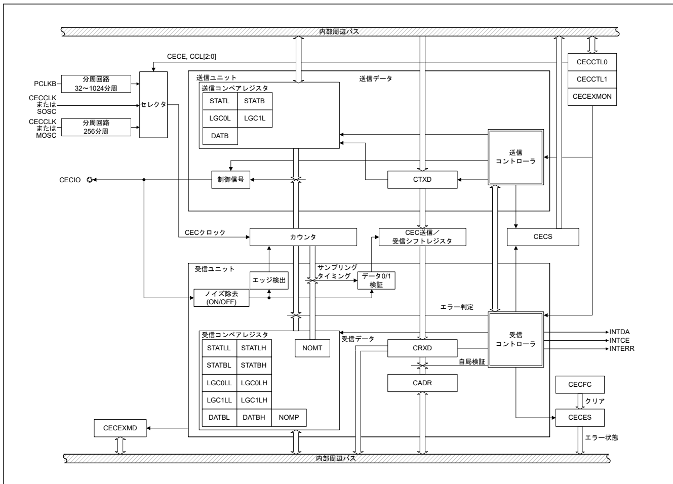
図 37.1 CEC のブロック図
