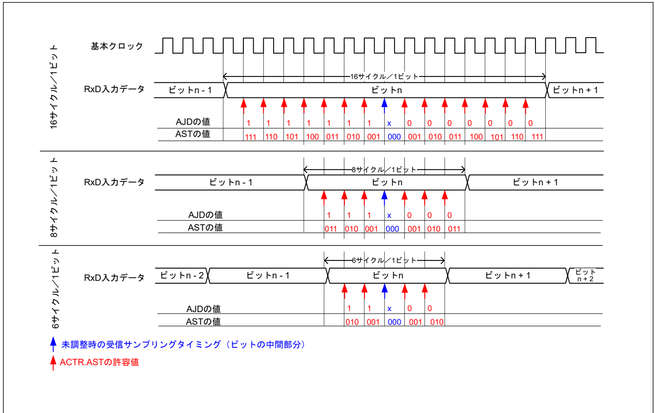
図 30.34 受信サンプリングタイミングの調整動作の概要 (内部クロックを使用した調歩同期式モード)
