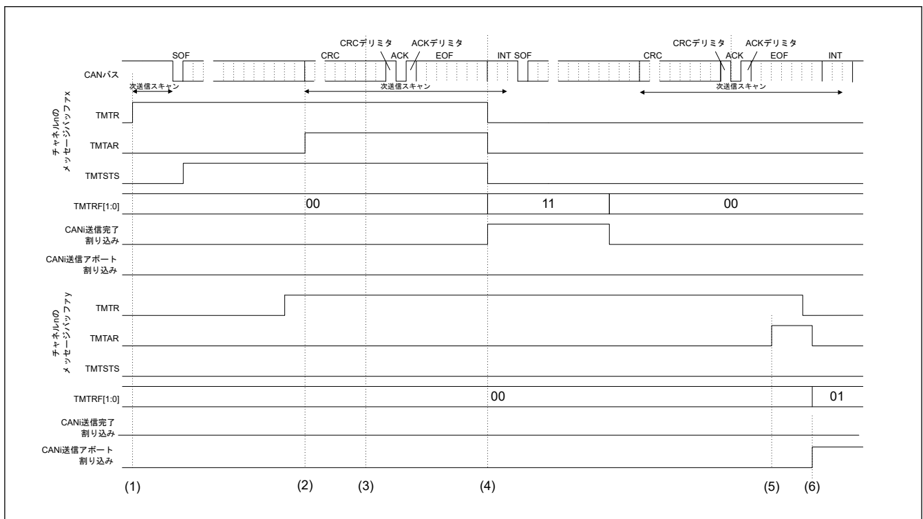
図 32.43 送信アボートの要求およびフラグビットのタイミング
