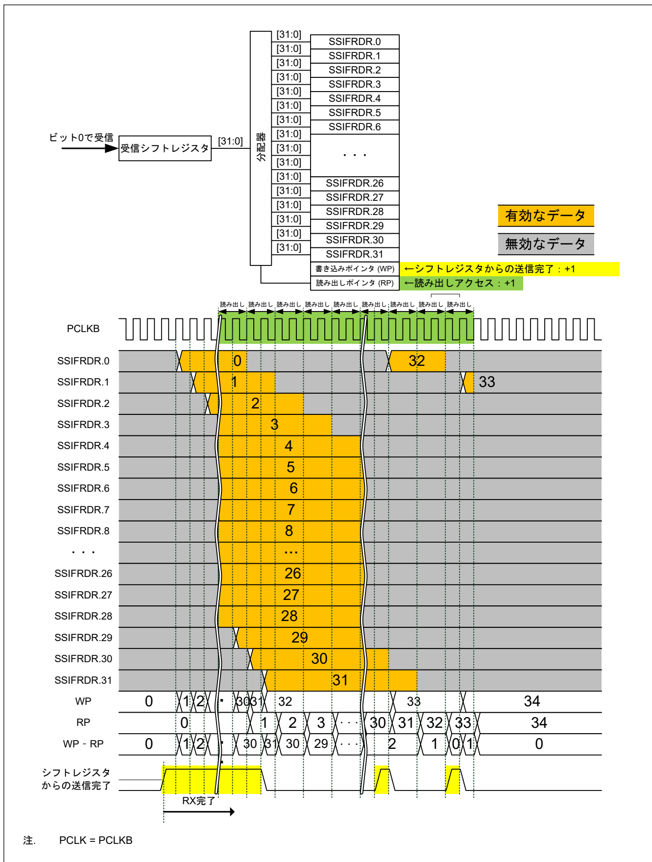
図 38.32 受信 FIFO データレジスタと受信シフトレジスタの構成、および FIFO の動作例
