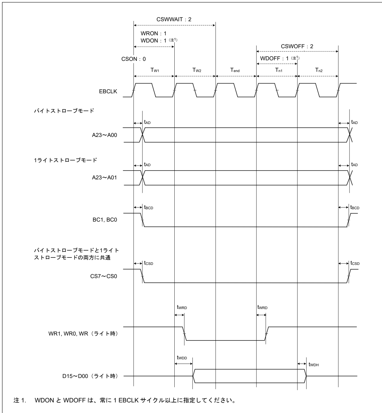
図 53.23 バスクロック同期を使用したノーマルライトサイクルの外部バスタイミング
