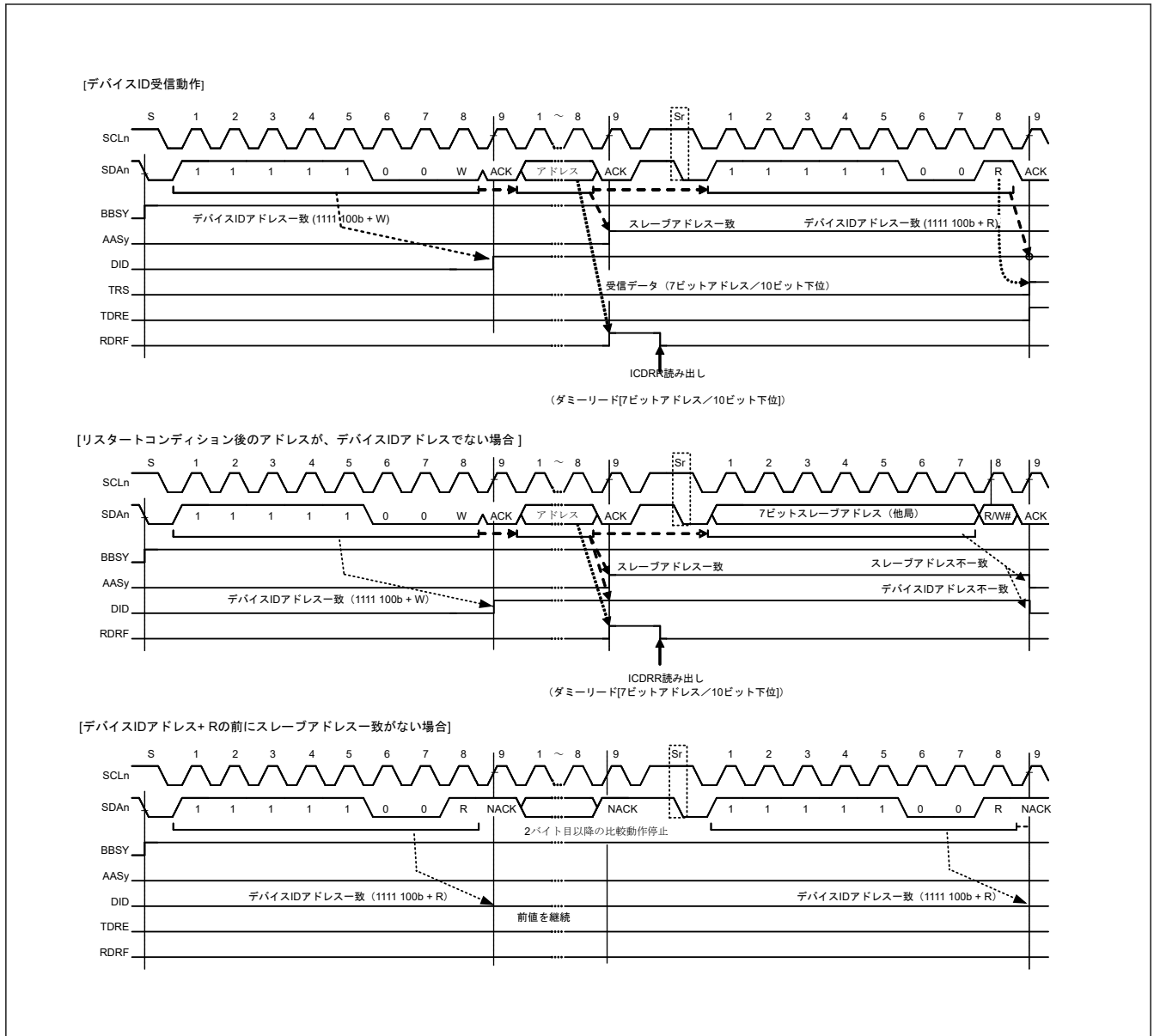
図 31.28 デバイス ID 受信時の AASn、DID フラグのセット/クリアタイミング
