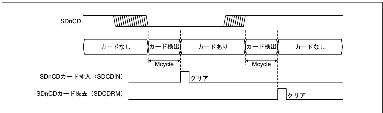
図 39.7 SDnCD によるカード検出例
