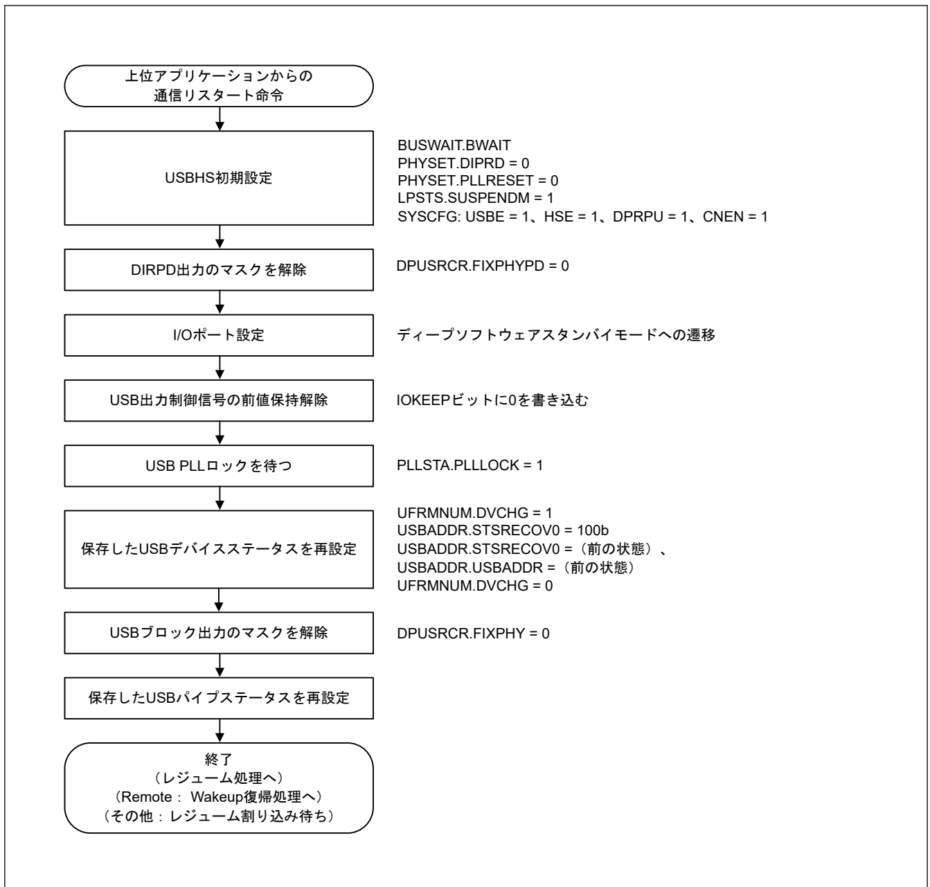
図 29.26 デバイスコントローラとしてディープソフトウェアスタンバイモードを解除する場合の USBHS 設定フロー (2)
