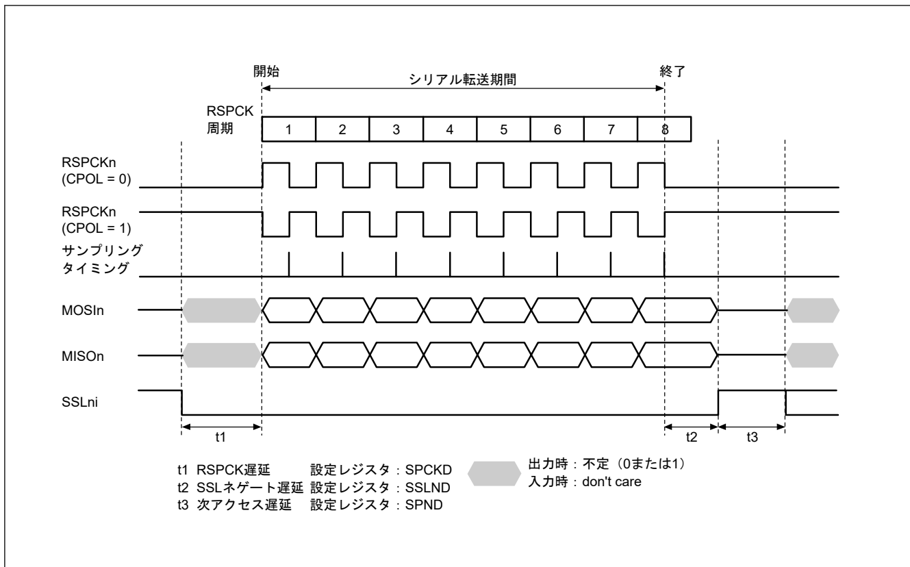
図 34.25 SPI 転送フォーマット (CPHA = 1 の場合)
