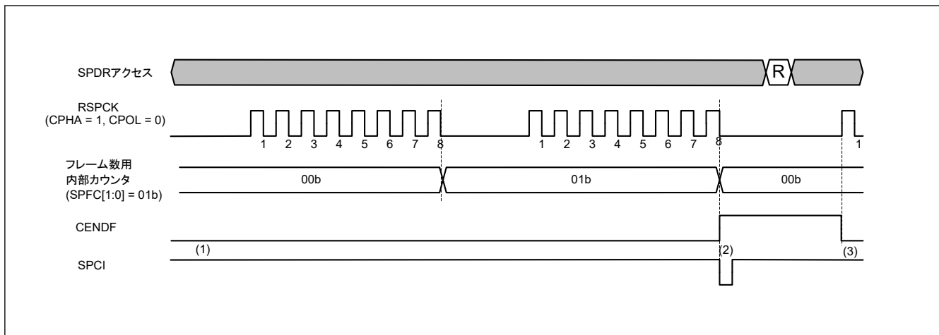
図 34.35 通信終了割り込み動作例 (クロック同期式動作時の受信のみスレープモード)
