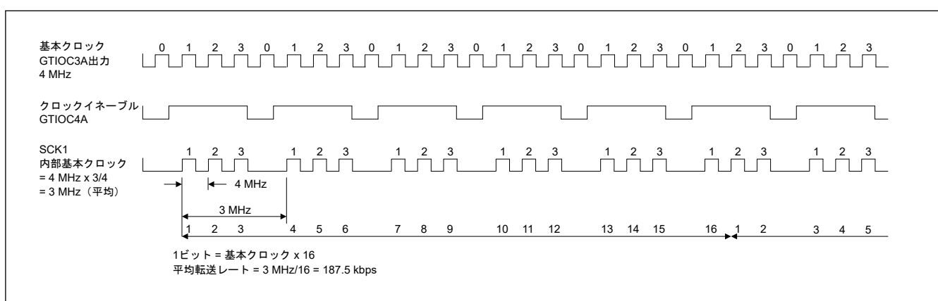
図 30.4 GPT クロック入力時の平均転送レート設定例
