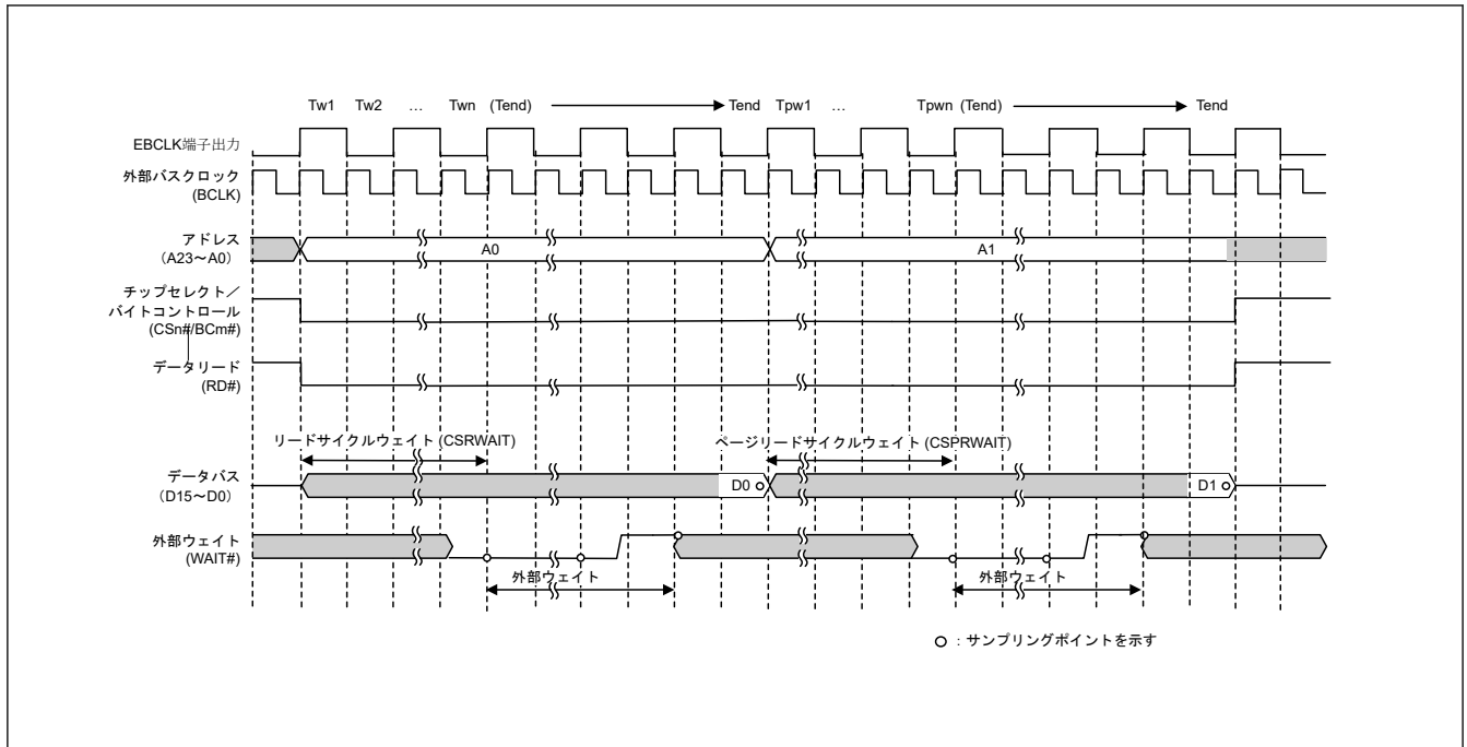
図 14.27 16 ビットバス空間に対するページリードアクセスの外部ウェイトタイミング例 (EBCLK 端子出力選択ビットで BCLK の 2 分周を選択した場合) (n = 0~7、m = 0、1)
