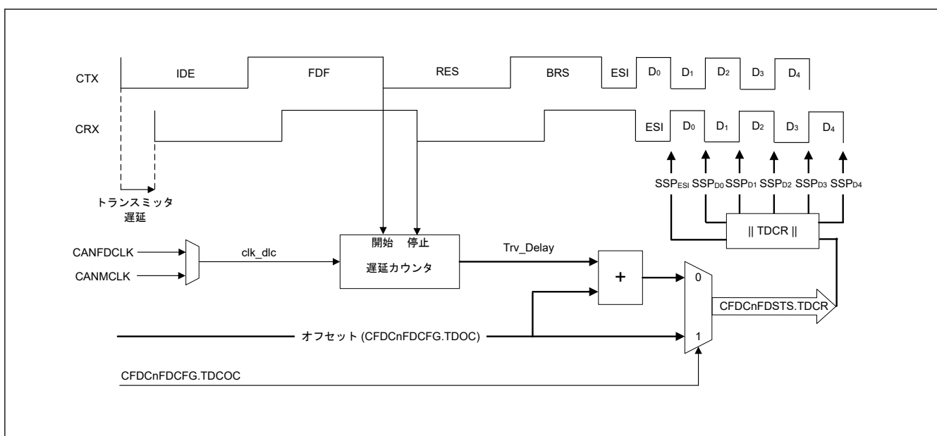
図 32.18 トランスミッタ遅延補償
