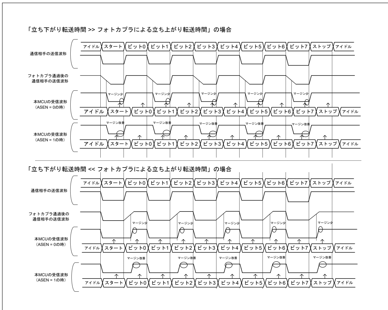
図 30.33 受信サンプリングタイミング調整機能による受信マージン向上の例
