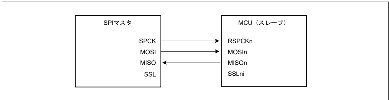
図 34.12 クロック同期式動作のマスタとスレーブの構成例 (MCU はスレーブ、CPHA = 1)
