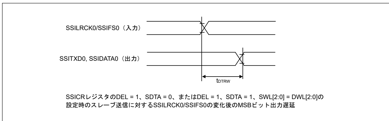
図 53.62 SSILRCK0/SSIFS0 変化時からの SSIE データ出力遅延
