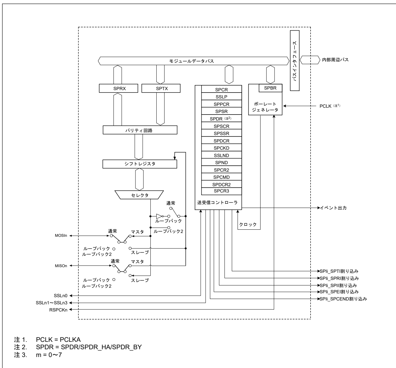
図 34.1 SPI のブロック図
