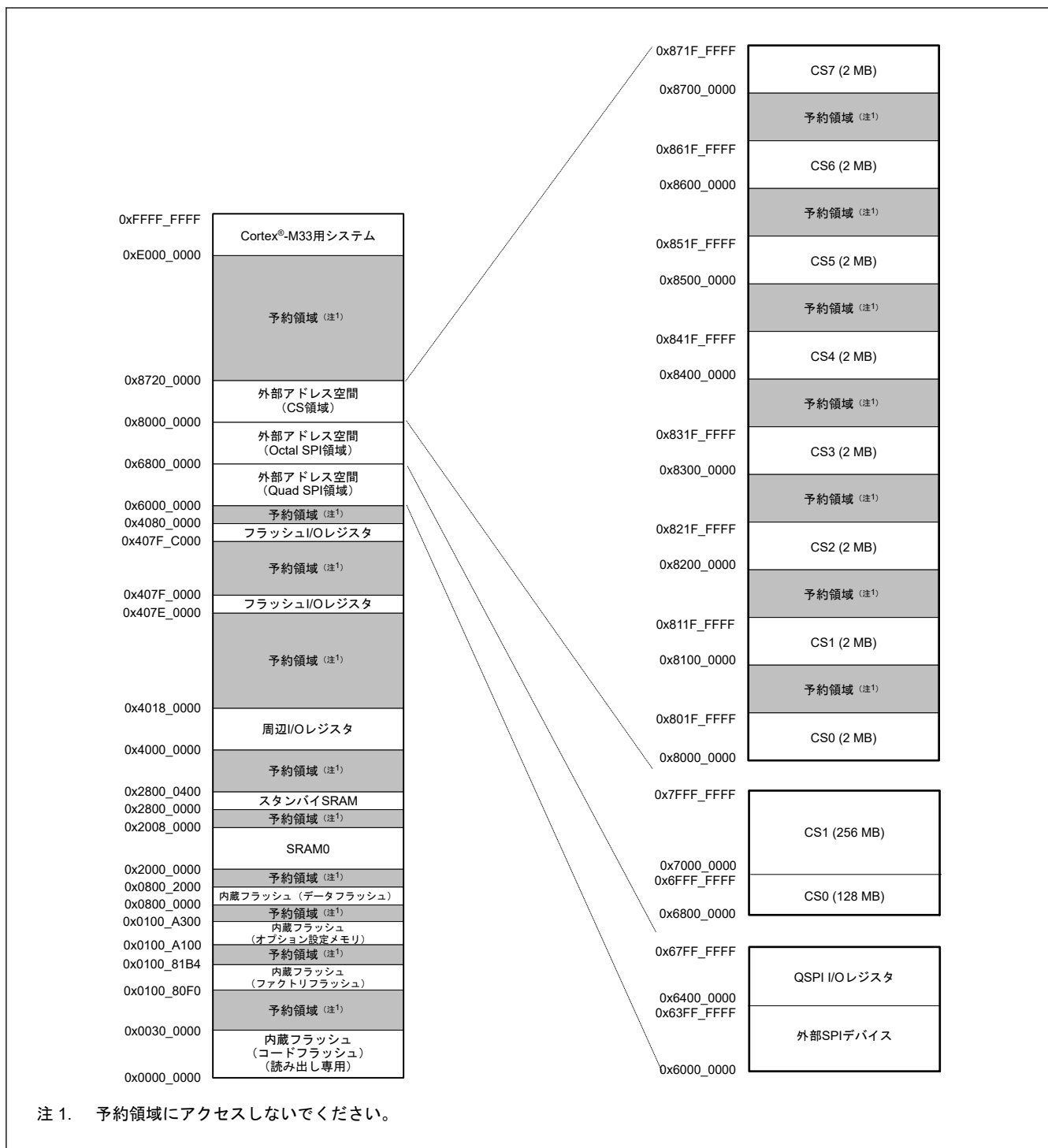
図 4.2 外部アドレス空間の対応関係 (144 ピン、100 ピン)
