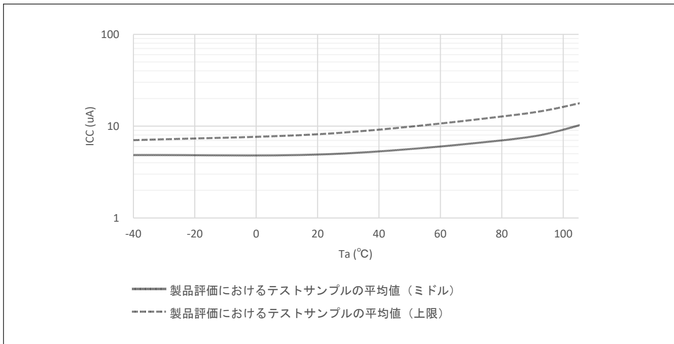
図 53.5 ディープソフトウェアスタンバイモード時の温度依存性、SRAM および USB レジューム検出部への電源供給なし、パワーオンリセット回路、低消費電力機能有効（参考データ）
