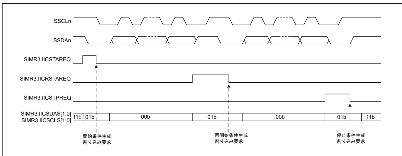
図 30.90 開始条件、再開条件、停止条件生成の動作タイミング
