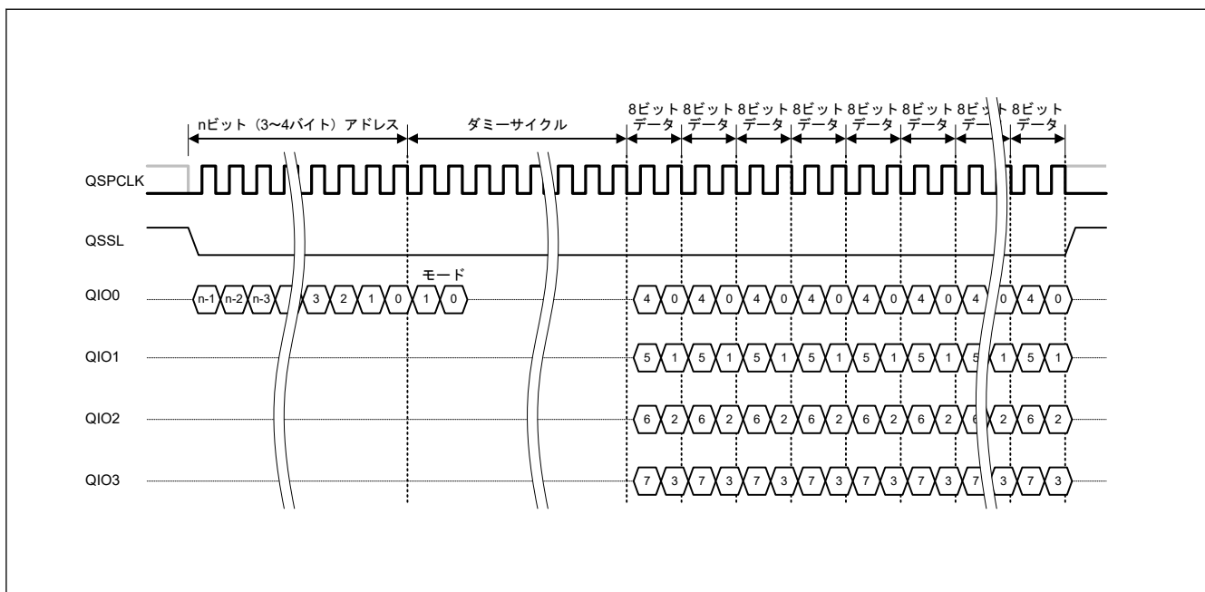
図 35.26 拡張 SPI プロトコルでの XIP モードファストリード Quad 出力バスサイクル
