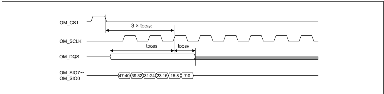
図 53.56 DQS リフレッシュ入力タイミング (OctaRAM™読み出し/書き込み)
