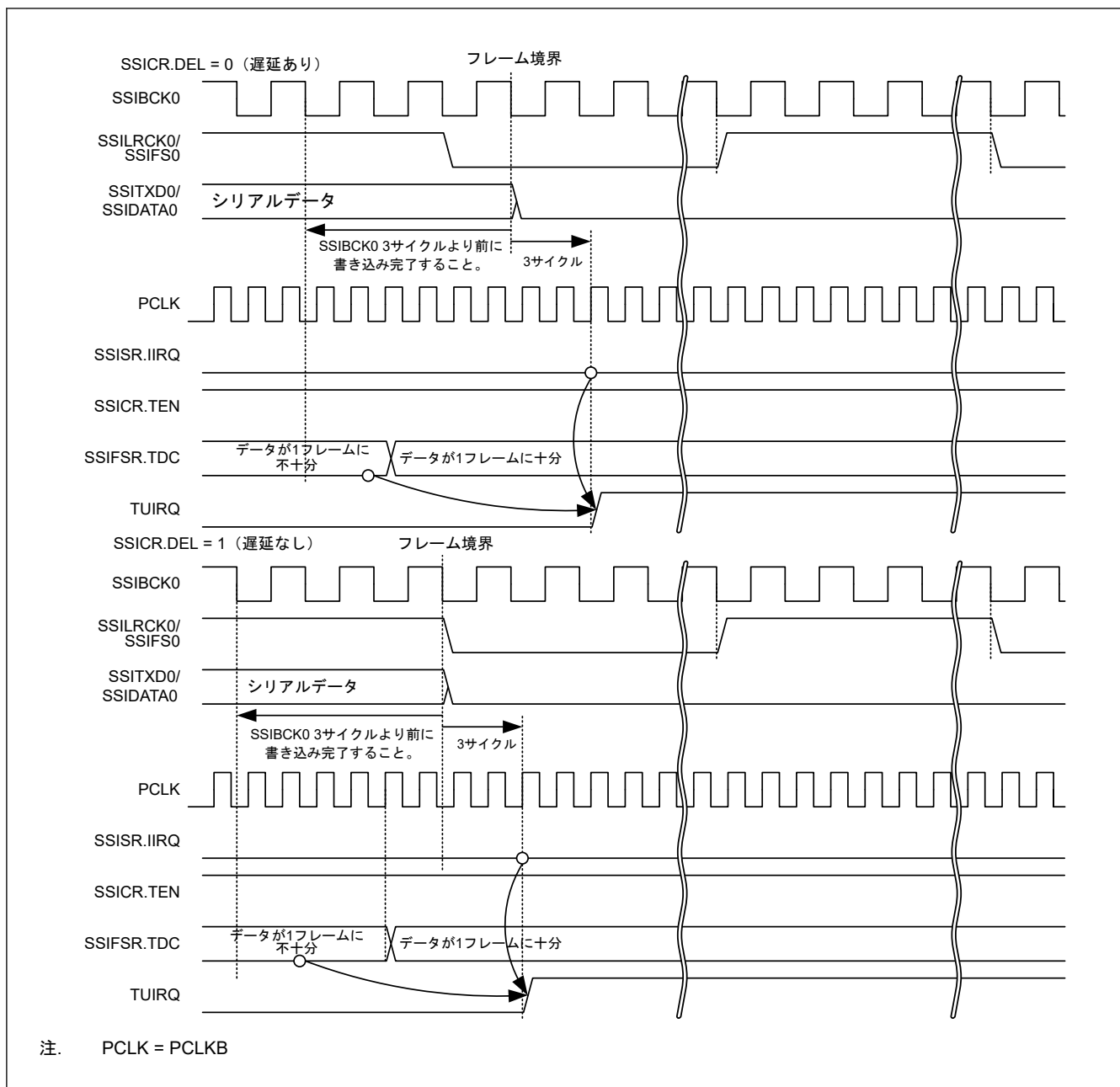
図 38.20 TUIRQ 設定タイミング (通信継続時)
