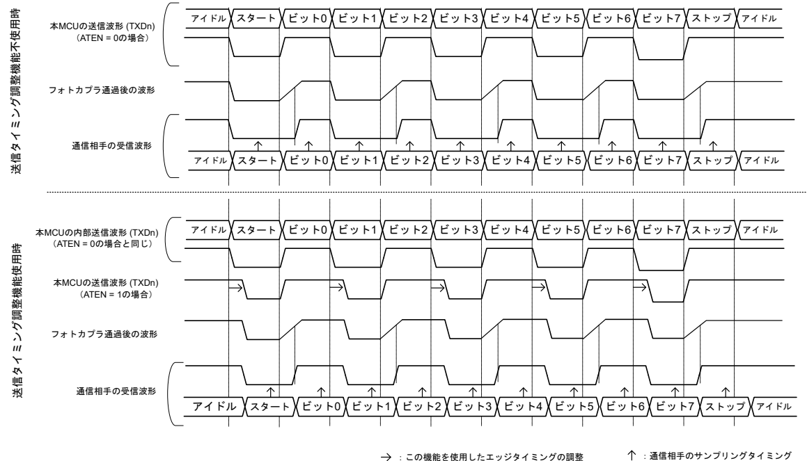
図 30.37 フォトカプラを経由する送信波形の説明
