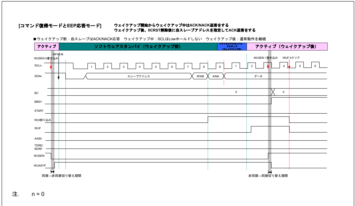
図 31.37 コマンドリカバリモードとEEP 応答モードのタイミング
