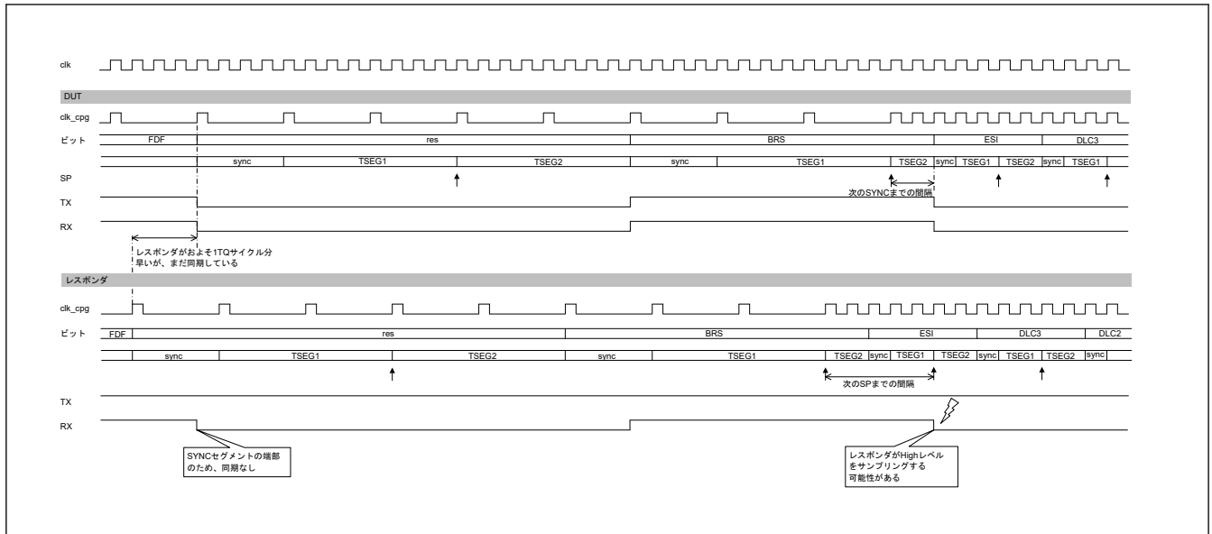
図 32.21 2つのCANノード間の同期ズレ
