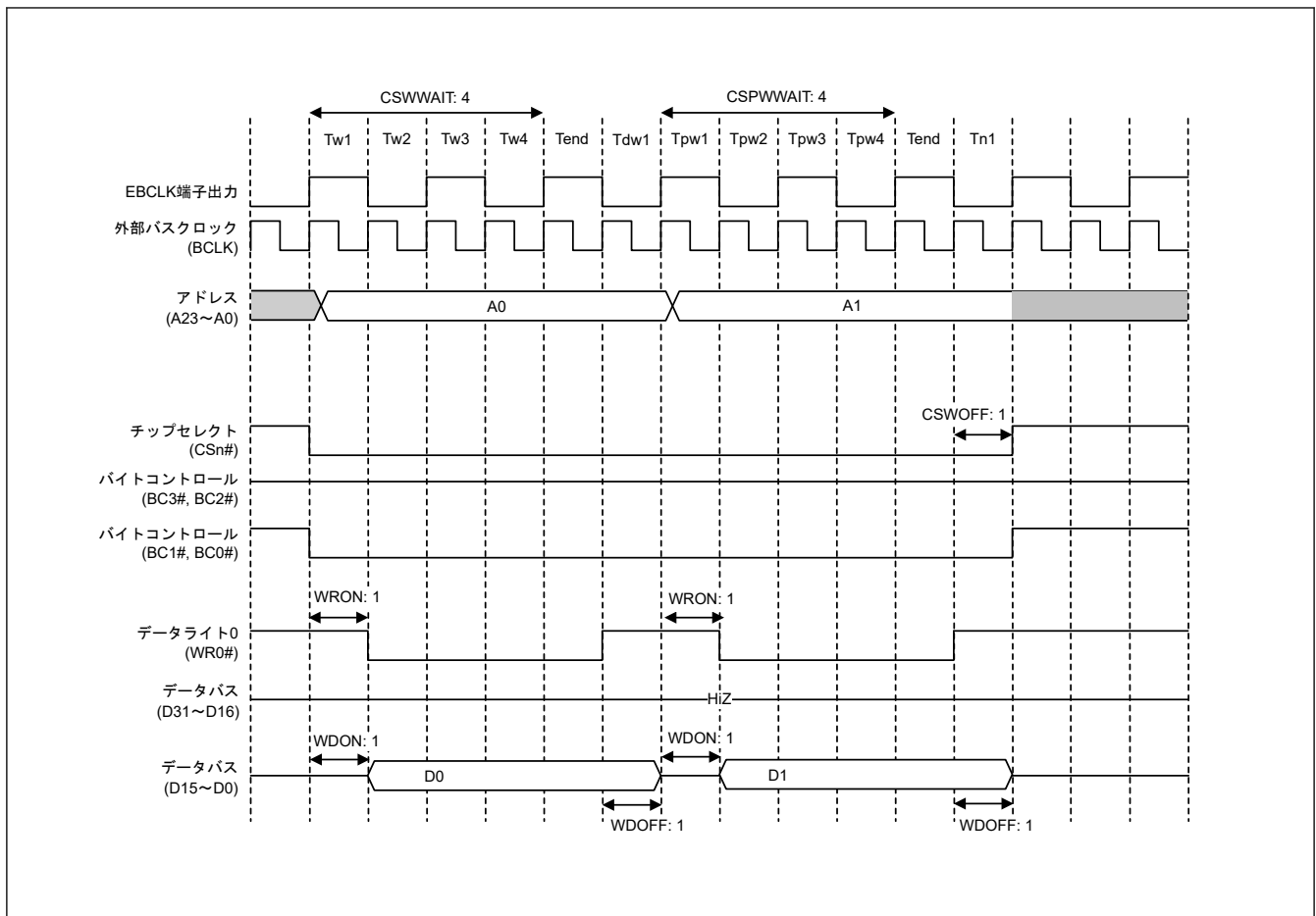
図 14.22 ページライトアクセスの動作例 (EBCLK 端子出力選択ビットで BCLK の 2 分周を設定した場合、および 1 転送要求に対して 2 回バスアクセスが発生する場合、1 ライトストローブモード時) ( n = 0 \sim 7 )
