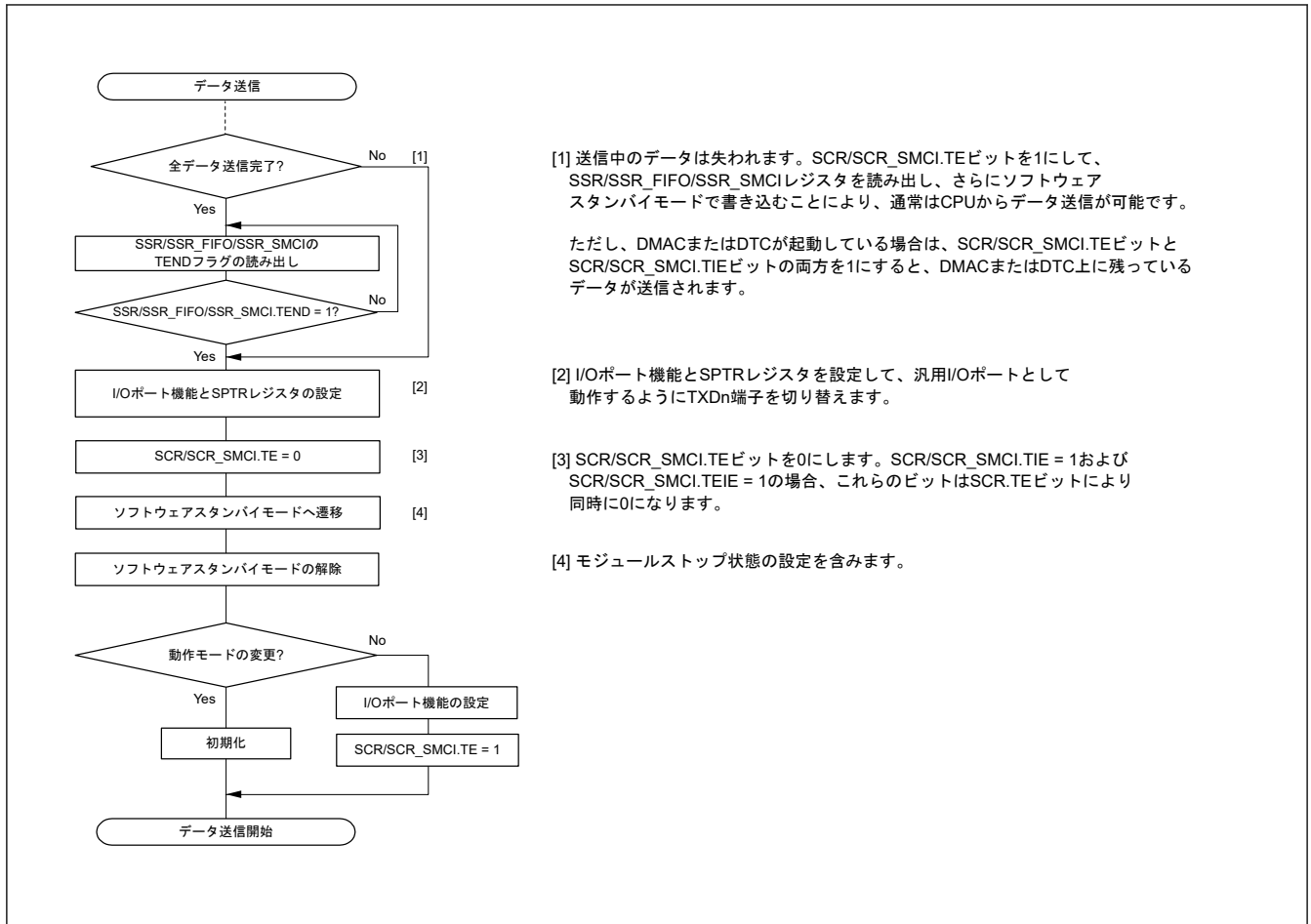
図 30.118 送信中にソフトウェアスタンバイモードへ遷移する場合のフローチャート例
