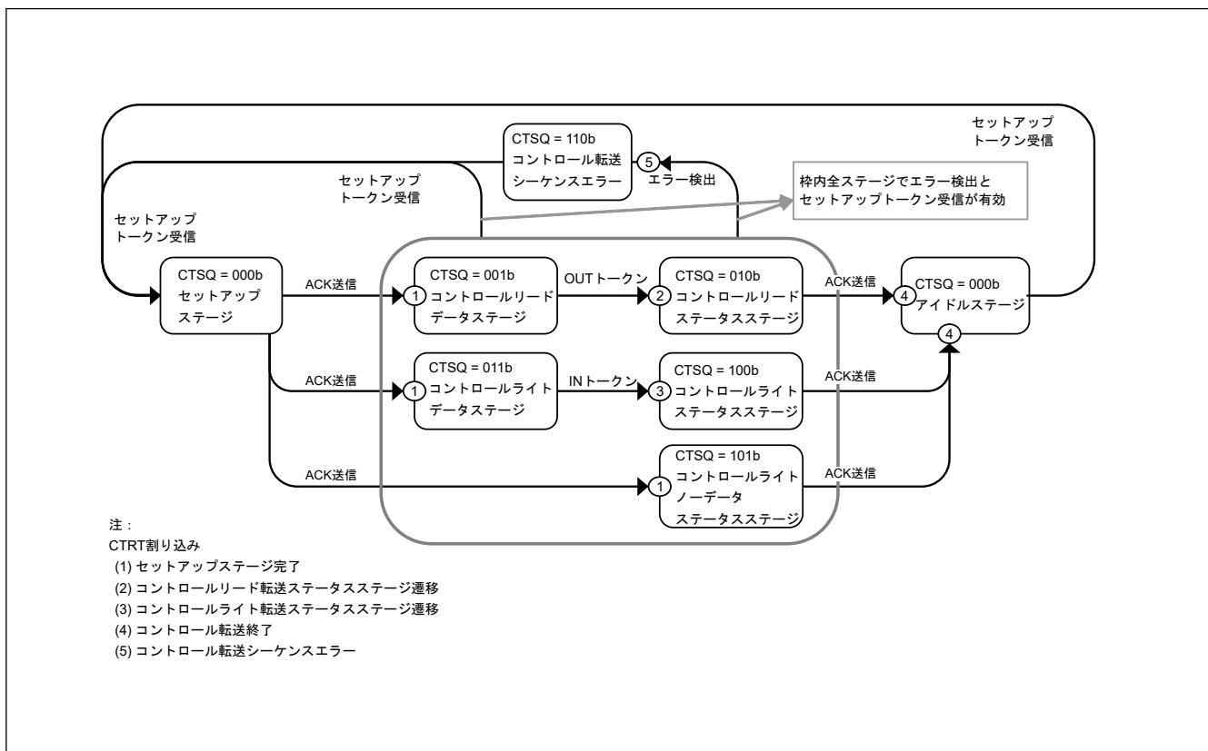
図 29.9 コントロール転送ステージの遷移
