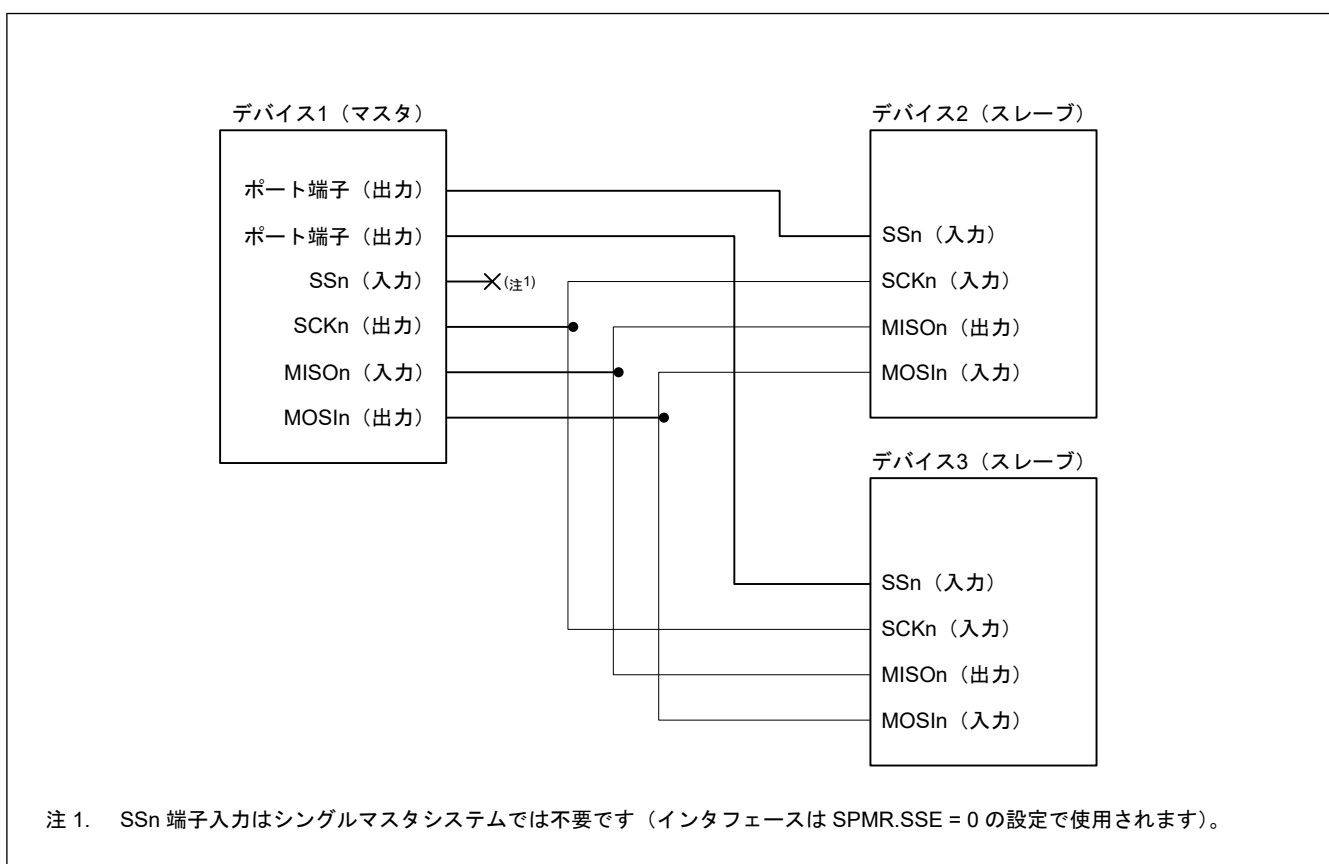
図 30.98 簡易 SPI モードでの接続例 (シングルマスタ時、SPMR.SSE ビット = 0)
