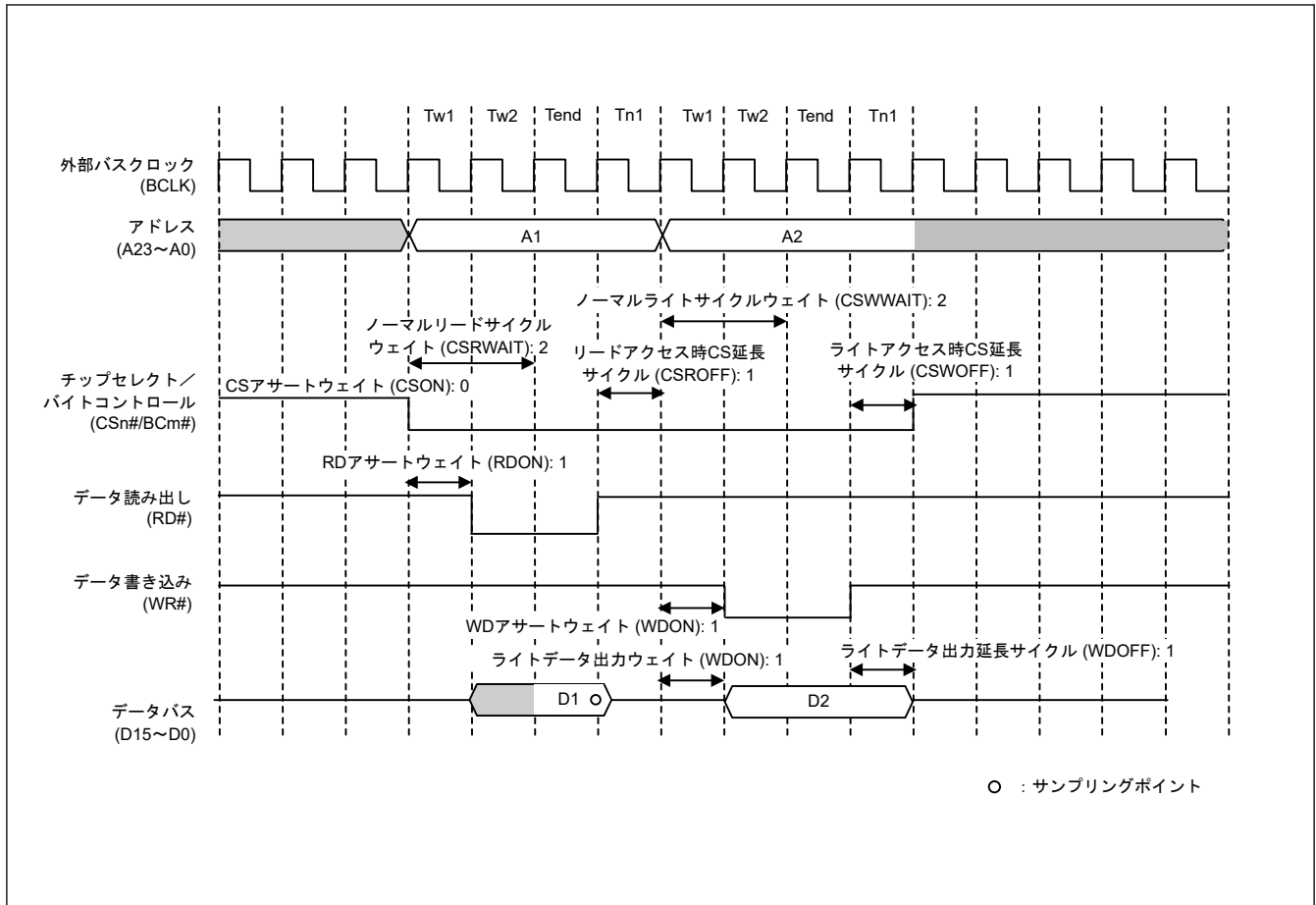
図 14.9 ノーマルアクセスの動作例 (読み出し、書き込み) (n = 0~7, m = 0~1)
