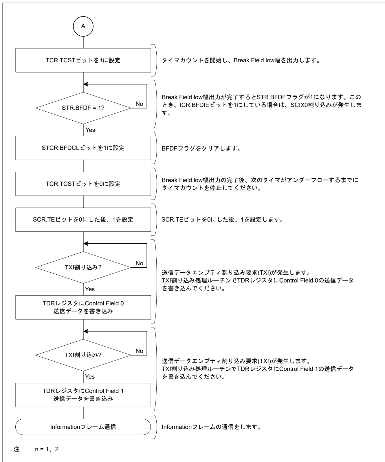
図 30.104 Start Frame 送信フローチャート例 (2/2)
