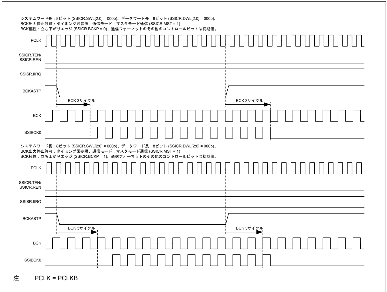
図 38.34 BCKASTP ビットの動作例 (アイドル状態の場合)
