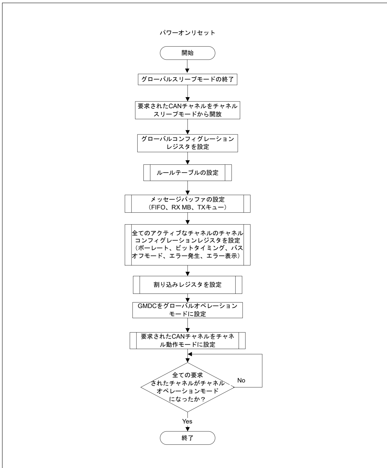
図 32.23 ハードウェアリセット後の構成手順
