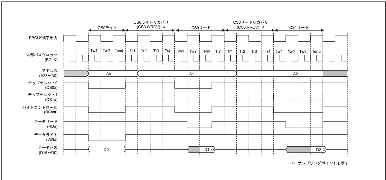
図 14.34 EBCLK 端子出力選択ビットで BCLK の 2 分周を選択した場合のリカバリサイクルの動作例（セパレートバスインタフェースによるノーマルアクセスの場合）(m = 0~1)
