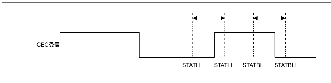
図 37.12 スタートビットの受信タイミング
