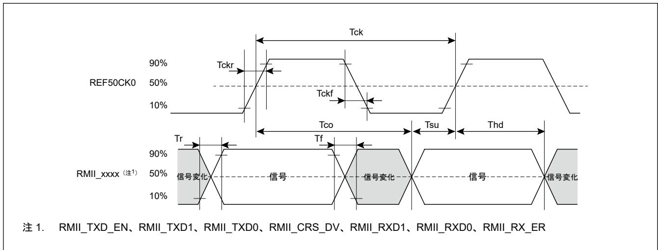
図 53.64 REF50CK0、RMII の信号タイミング
