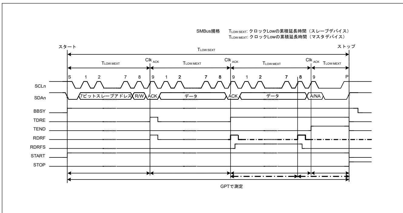
図 31.50 SMBus タイムアウト測定
