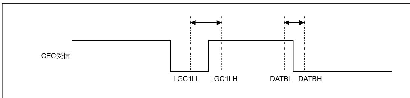
図 37.14 データビット (ロジカル 1) の受信タイミング
