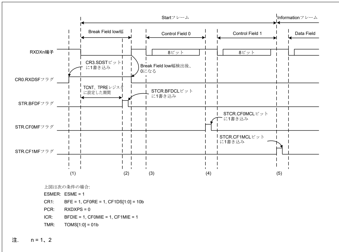
図 30.106 Start Frame 受信時の動作例
