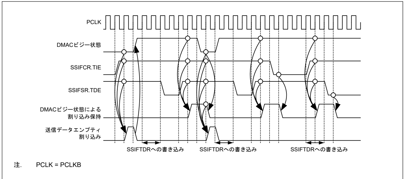
図 38.23 送信データエンプティ割り込みのタイミング
