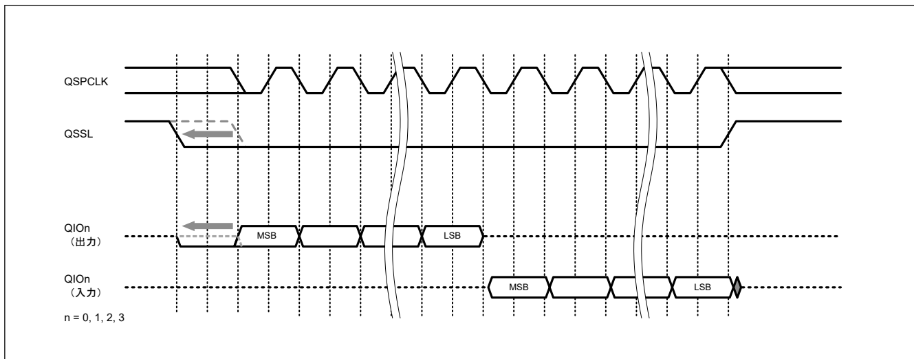
図 35.11 SFMSLD ビットを使用した QSSL 信号のセットアップ時間調整
