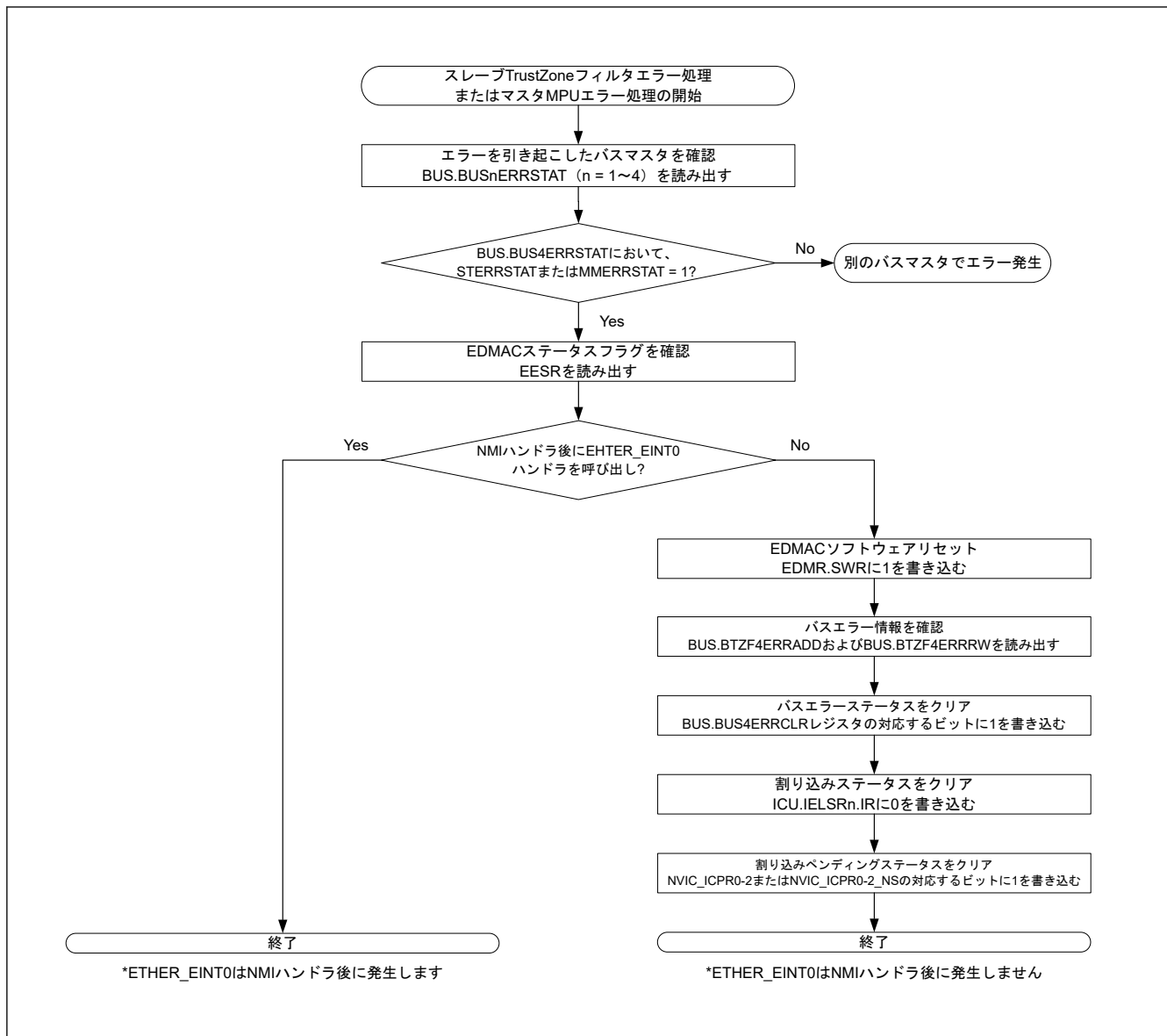
図 27.9 NMI ハンドラにおけるバス転送エラーの処理
