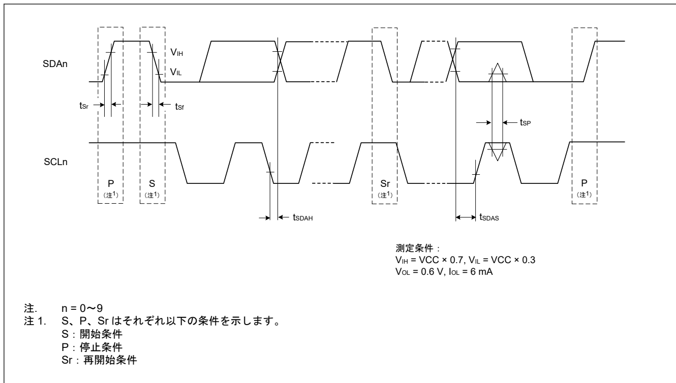
図 53.41 SCI 簡易 IIC モードタイミング
