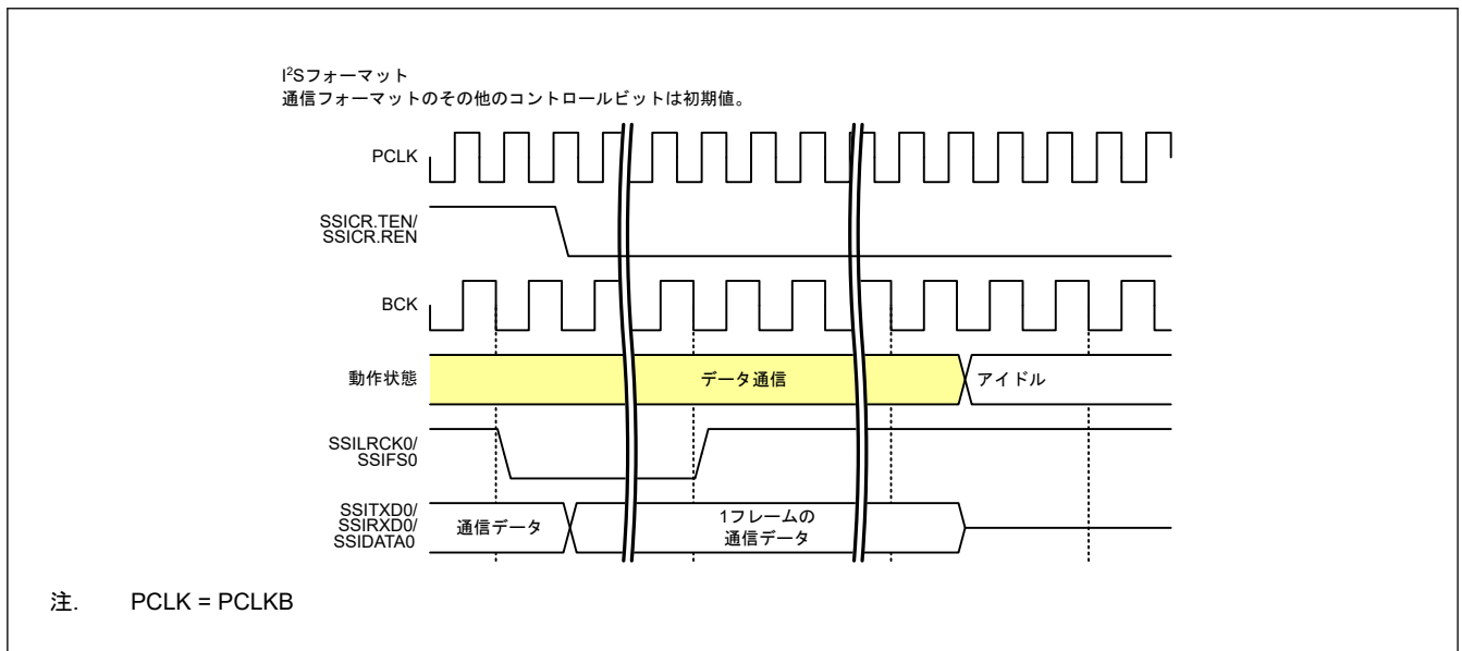
図 38.48 データ通信からの停止（パディングビットなし）
