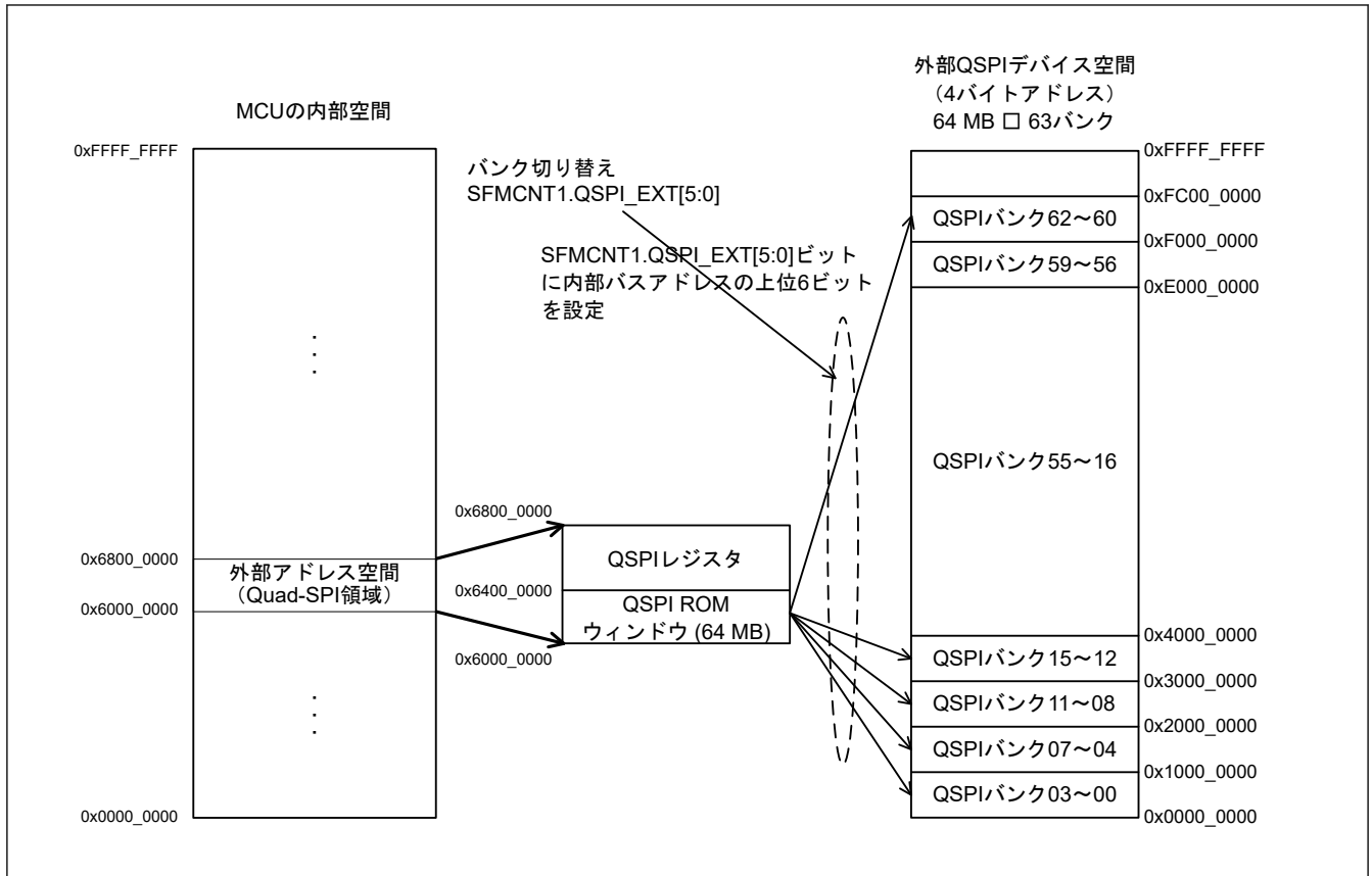
図 35.2 デフォルト領域設定およびメモリマップ
