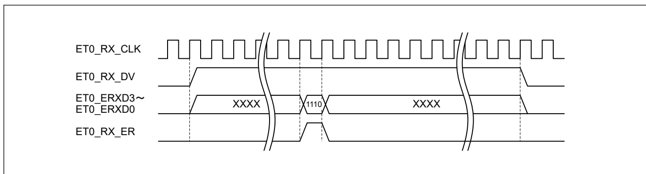
図 26.11 MII フレーム受信タイミング (不正キャリア通知時)
