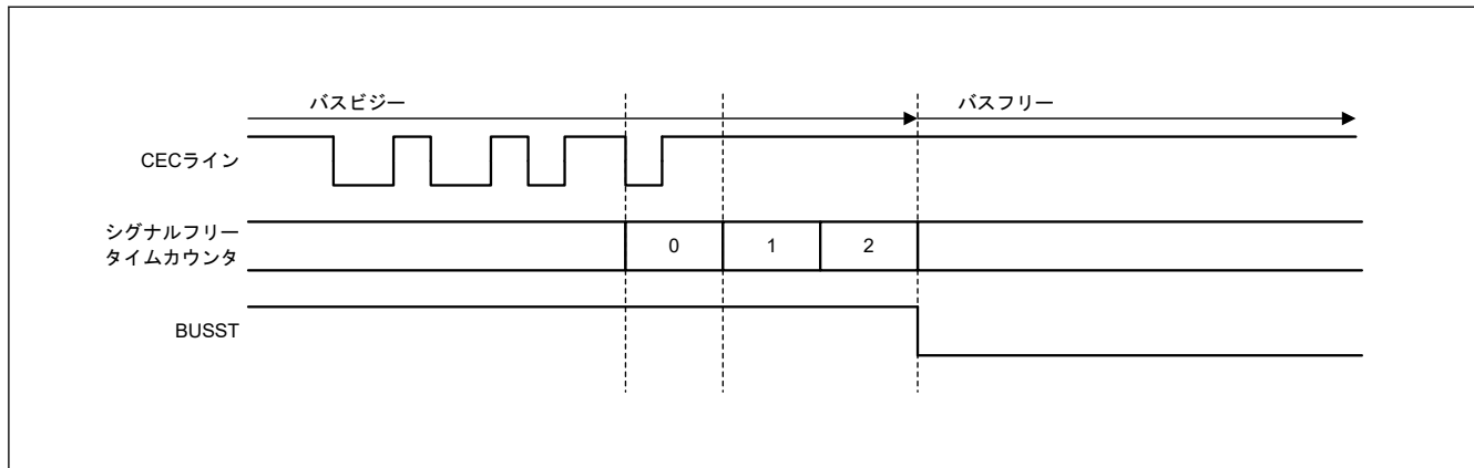
図 37.25 通信終了後、CECCTL1.SFT[1:0]ビットで設定したシグナルフリータイムを経過した場合のタイミング
