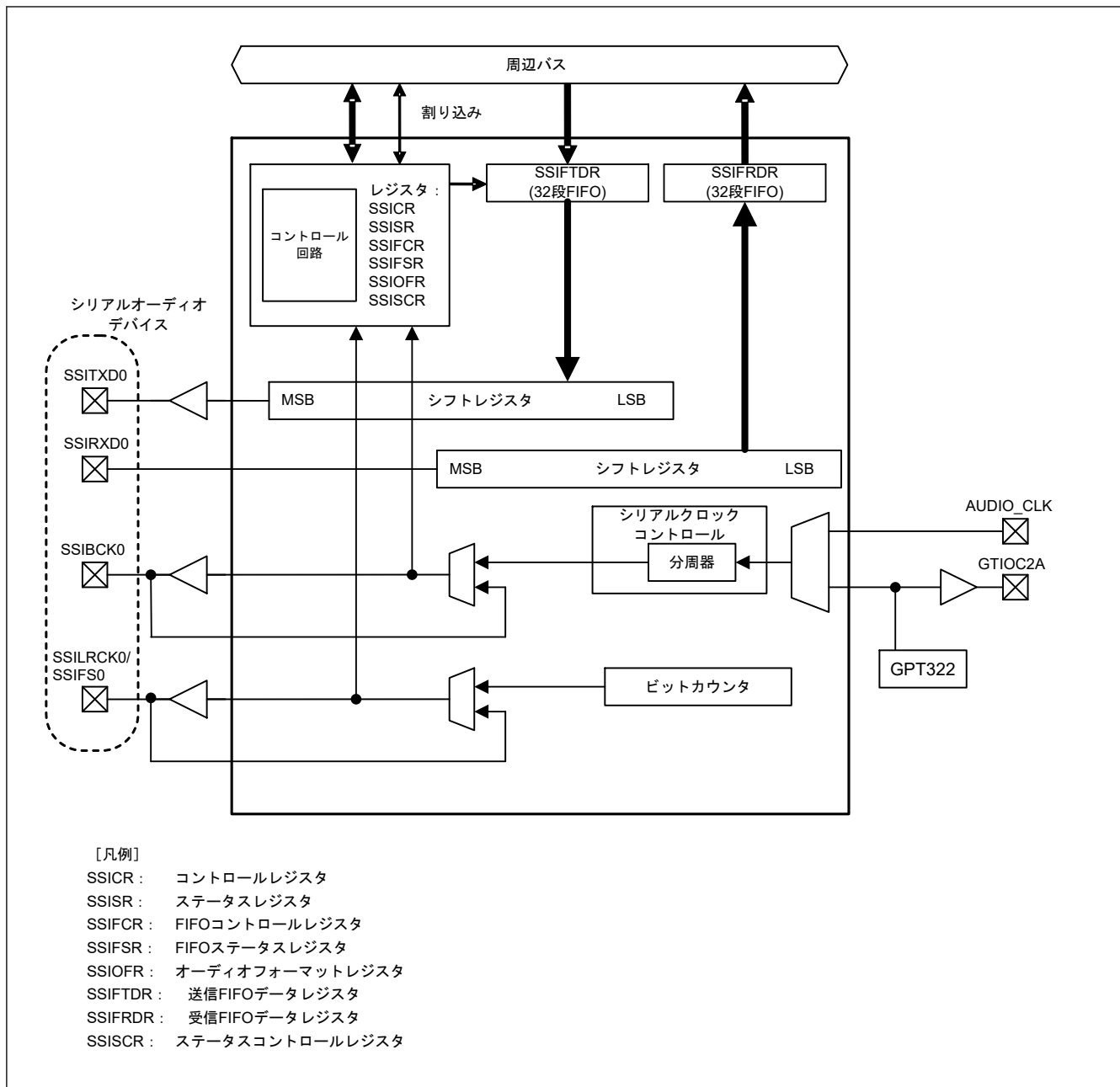
図 38.2 全二重通信の SSIE ブロック図
