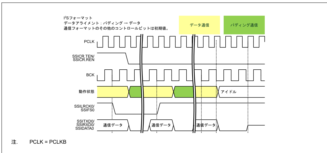
図 38.50 データ通信からの停止（パディングビットあり）
