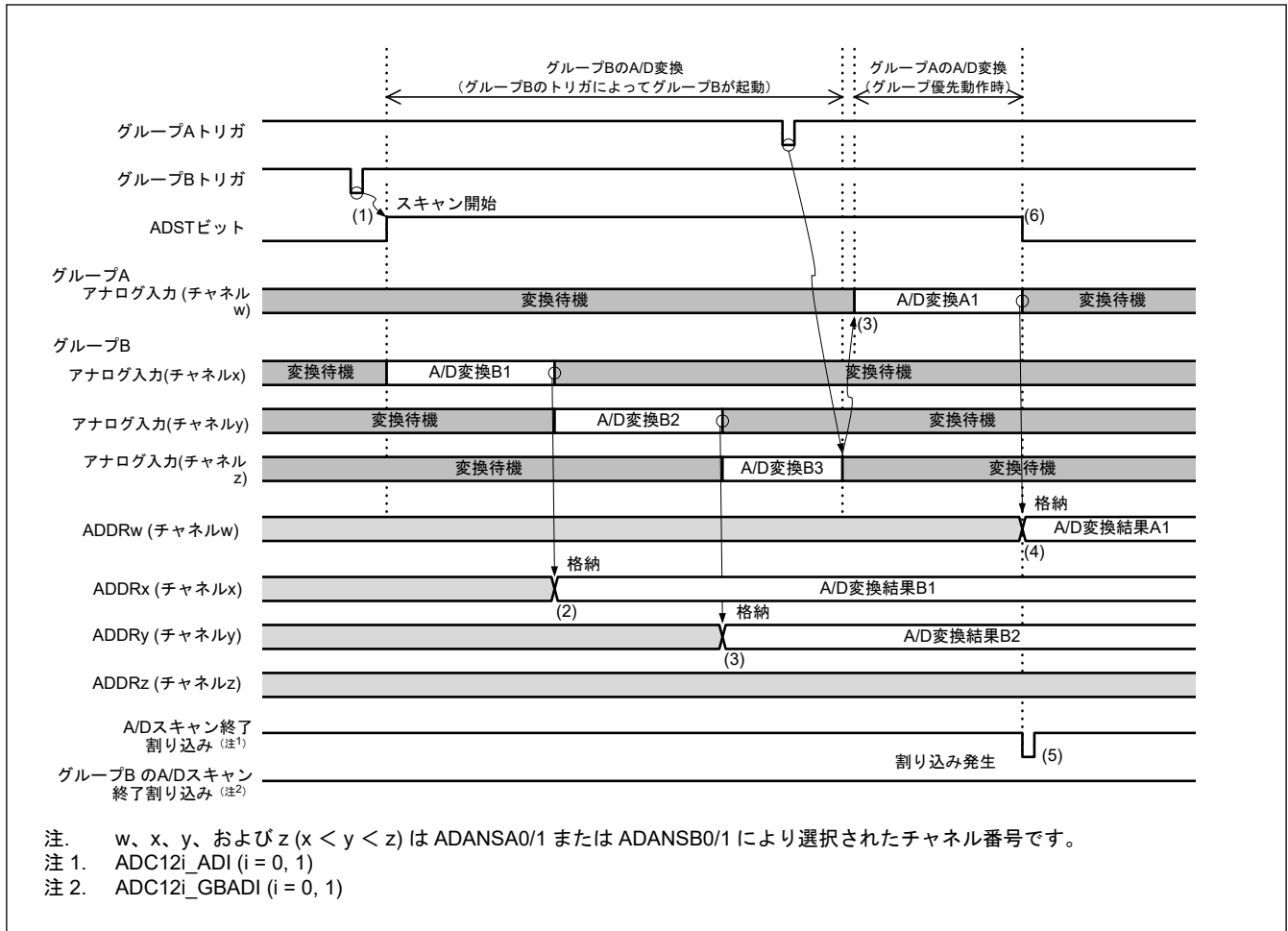
図 43.22 グループ優先動作の例 1-4 : グループ B スキャン中のグループ A トリガ入力、再スキャンなし (ADGSPCR.GBRSCN = 0、ADGSPCR.GBRP = 0、および ADGSPCR.LGRRS = 0 の場合)
