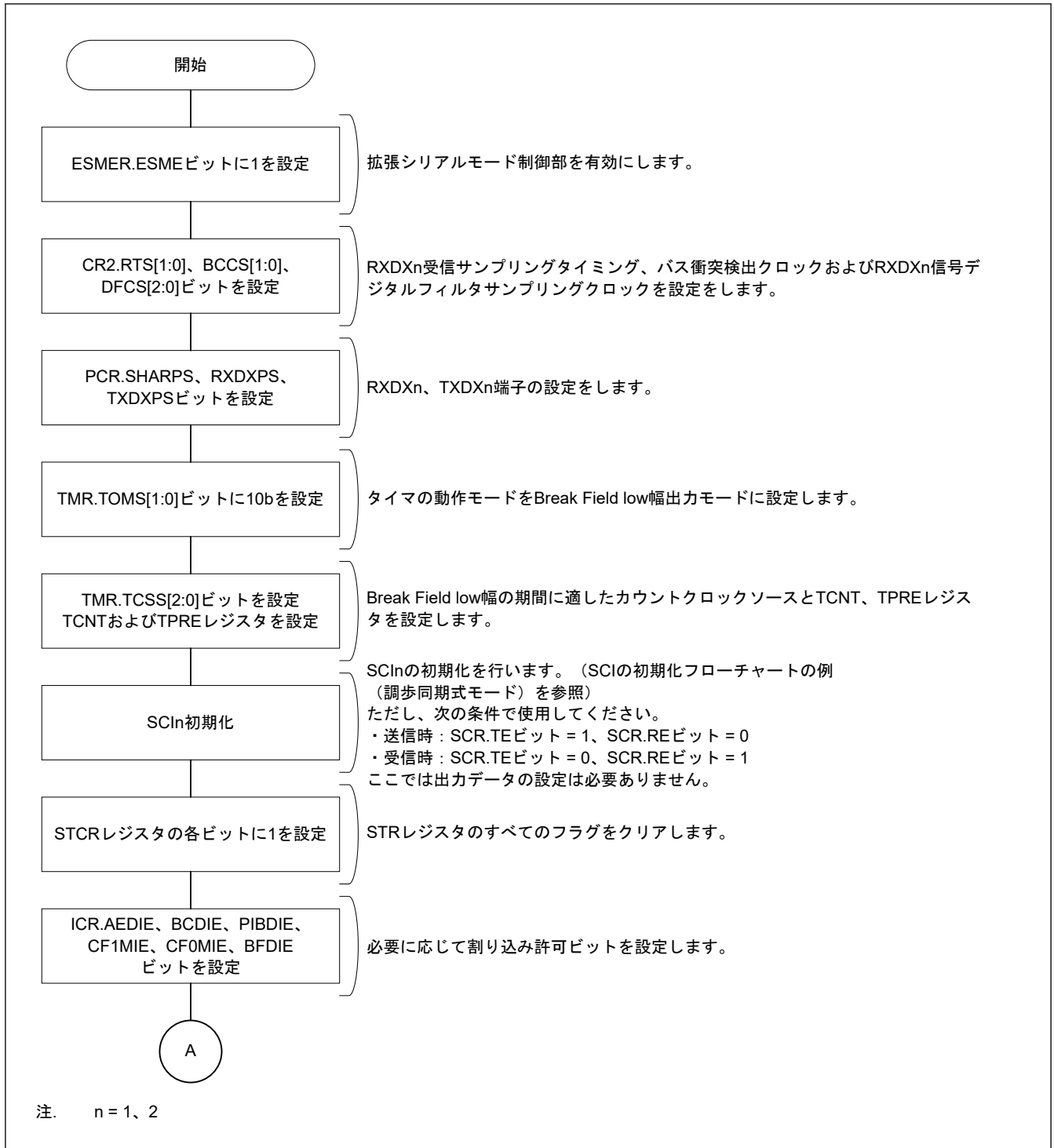
図 30.103 Start Frame 送信フローチャート例 (1/2)
