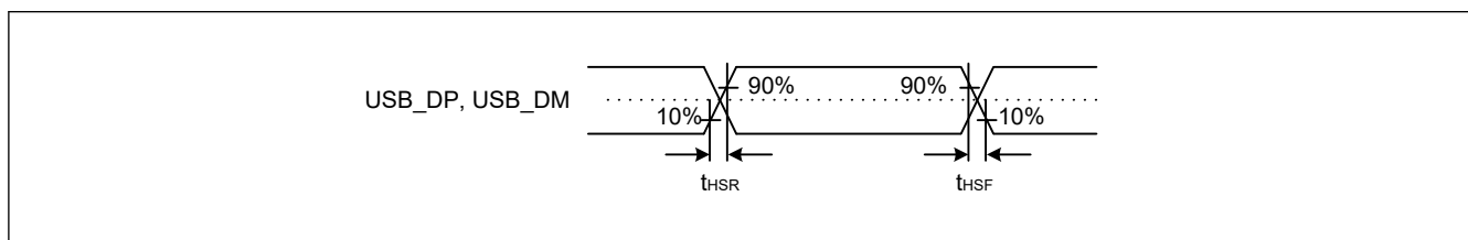
図 53.84 High-speed モードにおける USB_DP、USB_DM の出力タイミング
