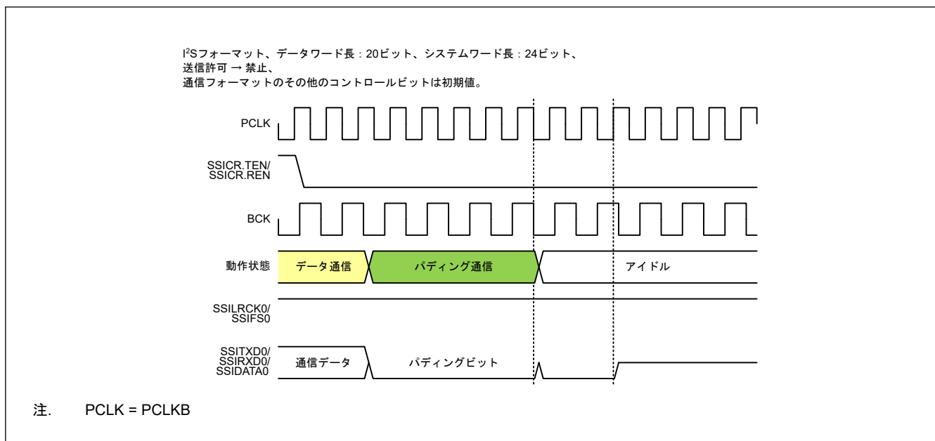
図 38.51 パディング通信からの停止
