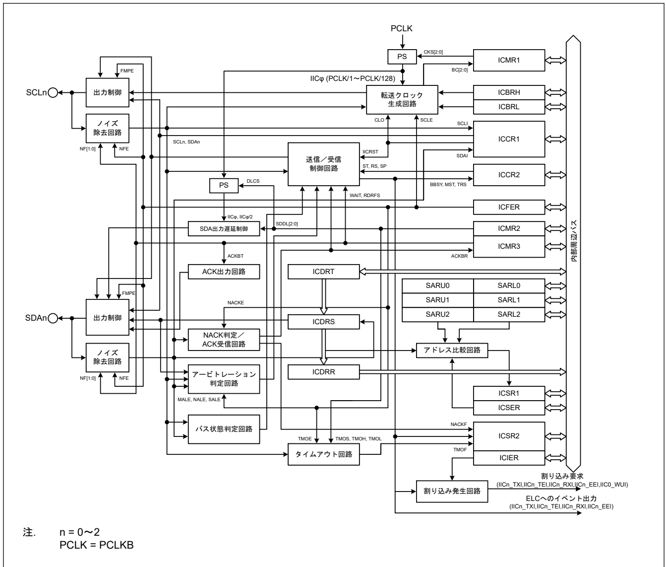
図 31.1 IIC のブロック図
