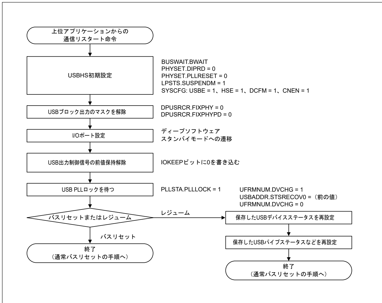
図 29.24 ホストコントローラとしてディープソフトウェアスタンバイモードを解除する場合の USBHS 設定フロー (2)
