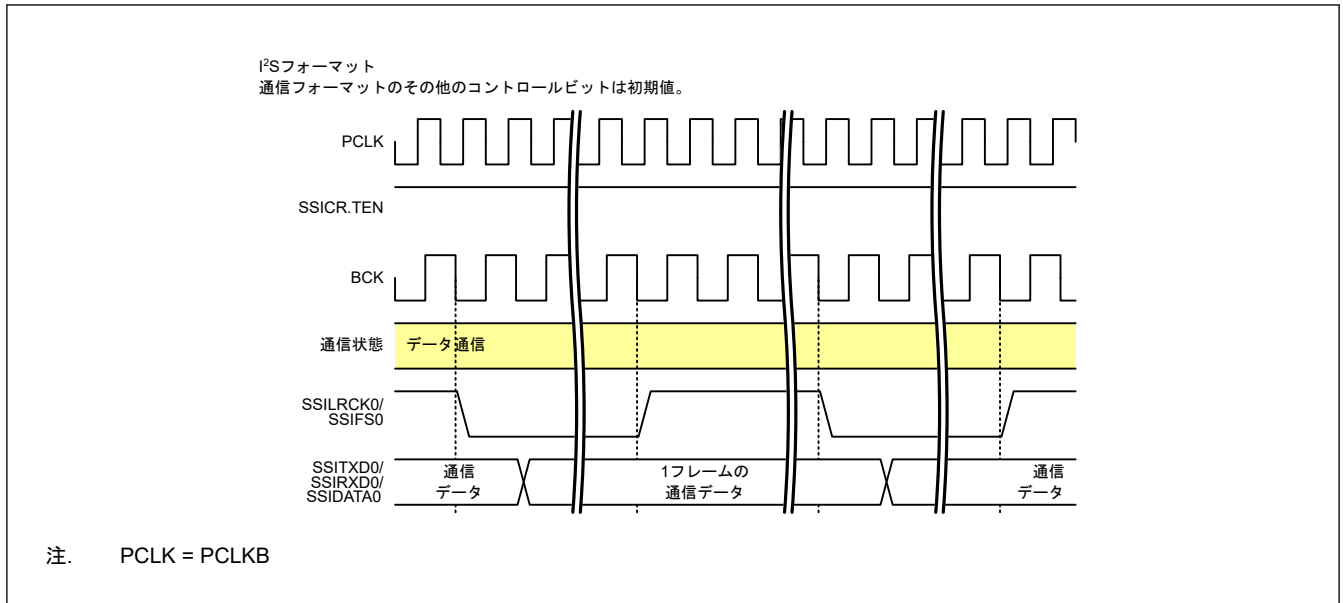
図 38.47 データ通信の継続
