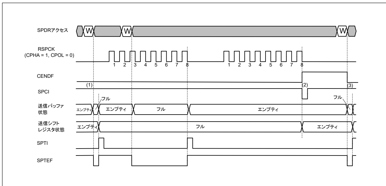
図 34.34 通信終了割り込み動作例（クロック同期式動作時の送受信／送信スレーブモード）
