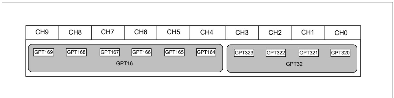
図 21.2 GPT チャンネルとモジュール名の関係
