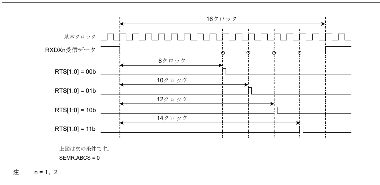
図 30.114 RXDXn 受信データサンプリングタイミング
