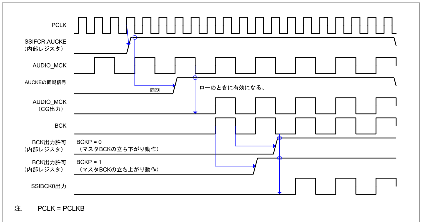
図 38.26 システムリセットからマスタモード通信開始までの動作のタイミング図
