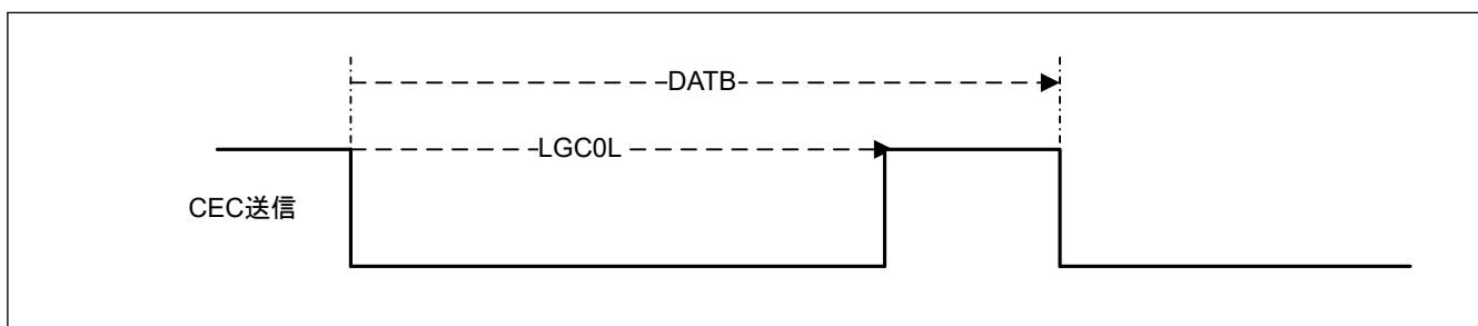
図 37.10 データビット (ロジカル 0) の出力波形
