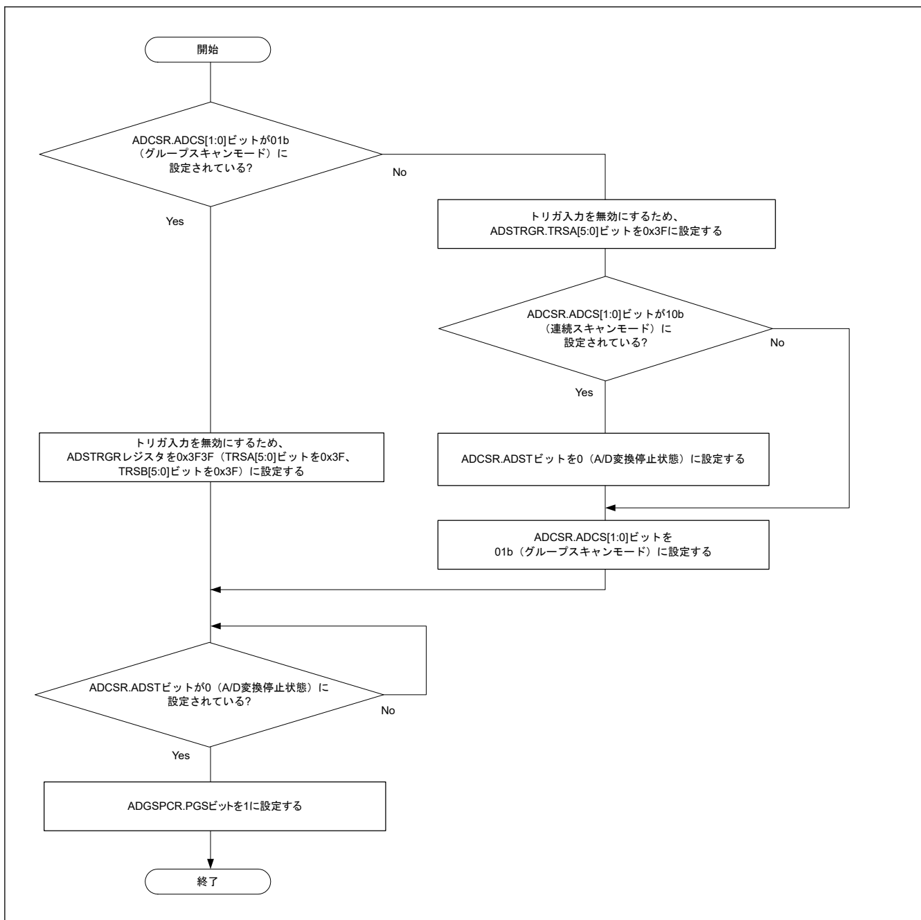
図 43.18 ADGSPCR.PGS ビット設定時のフローチャート
