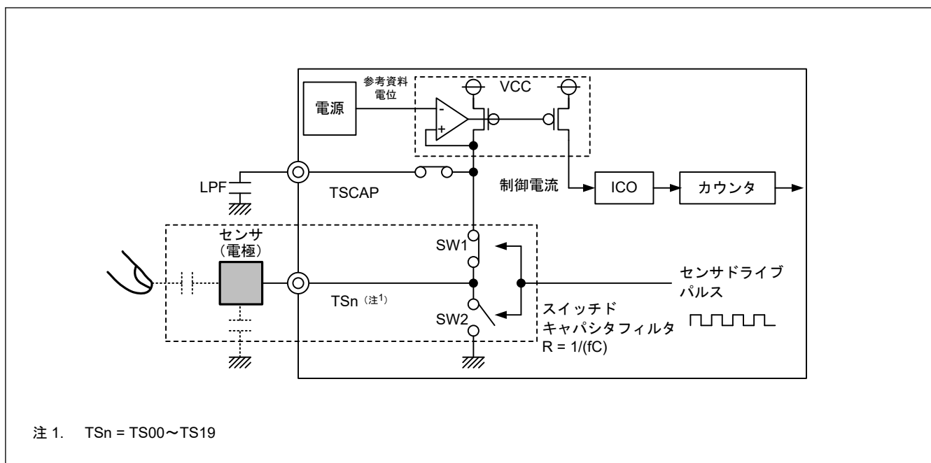
図 46.4 計測部回路
