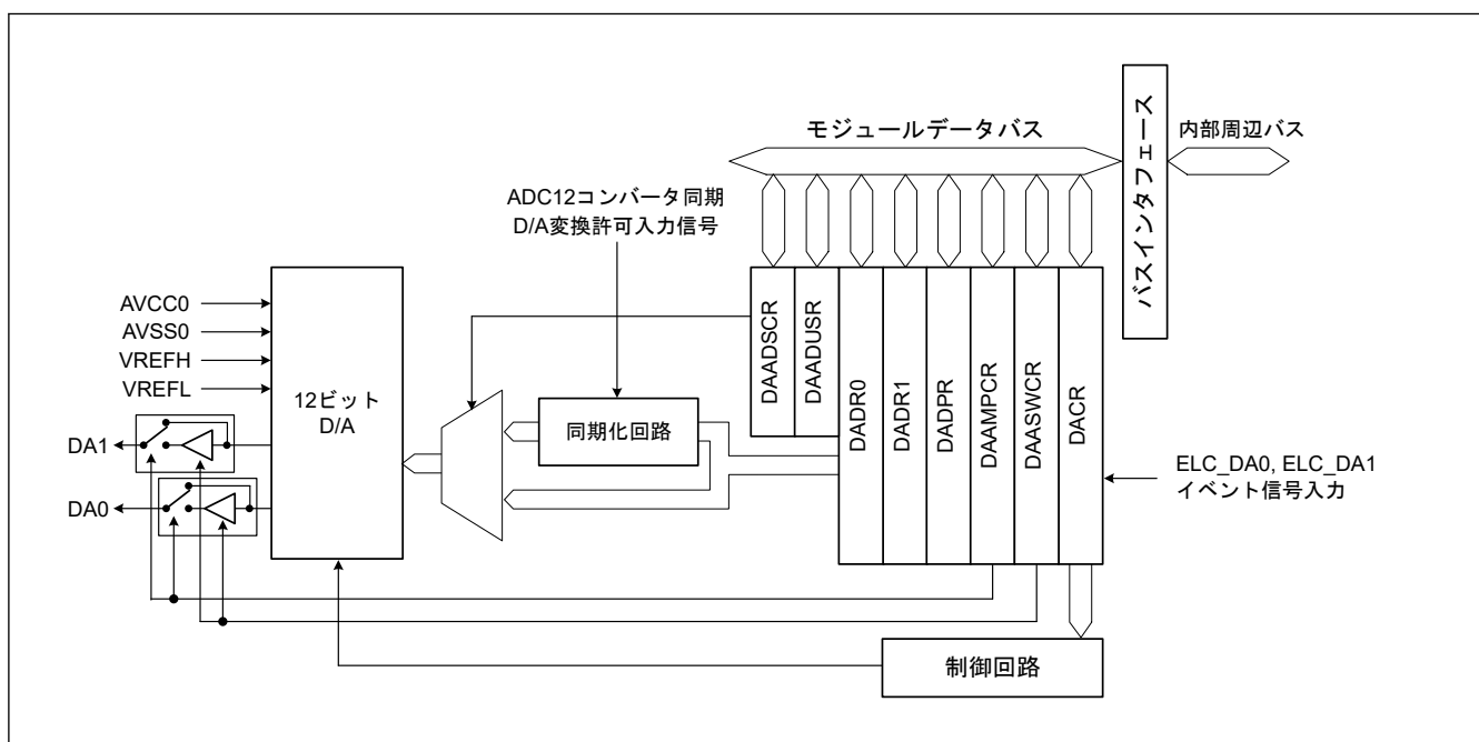
図 44.1 DAC12 のブロック図
