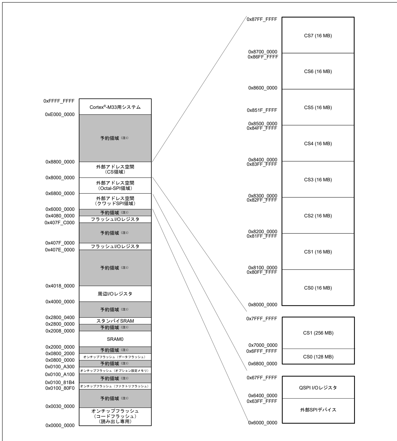
図 4.3 外部アドレス空間の対応関係 (176 ピン)
