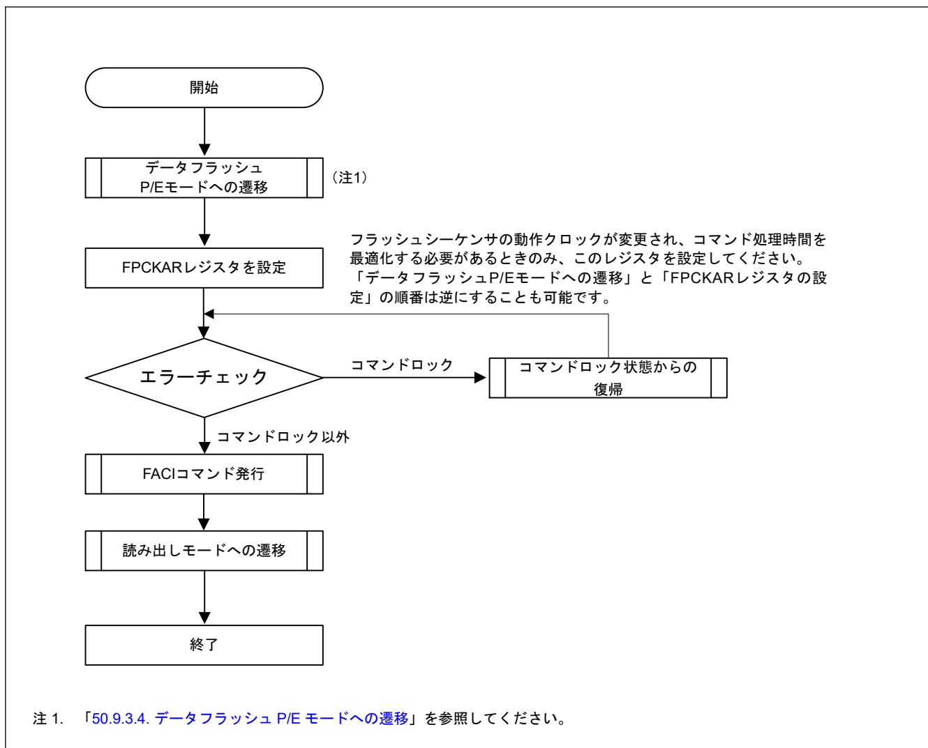
図 50.9 データフラッシュ P/E モードでのコマンド使用概要
