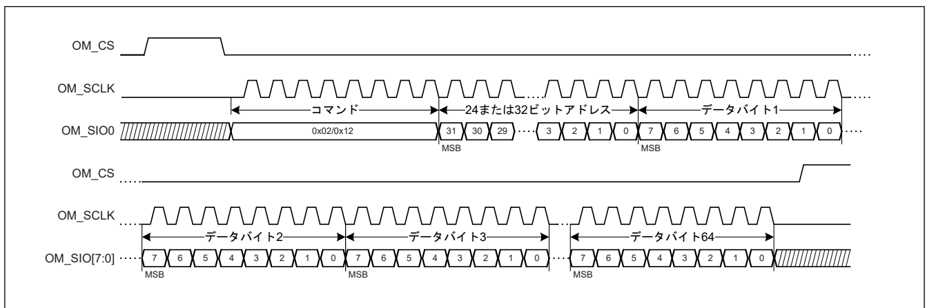
図 36.3 OctaFlash インタフェースでの書き込み動作の波形 (SPI モード)
