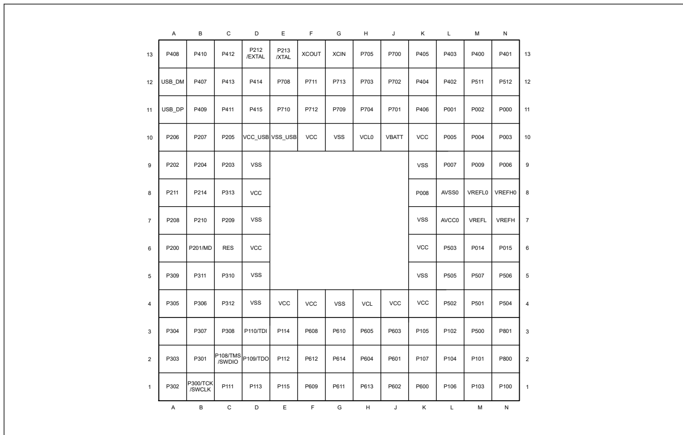
図 1.6 144 ピン BGA のピン配置
