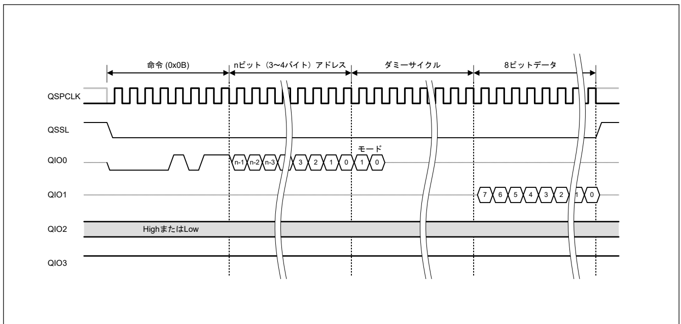
図 35.19 ファストリードバスサイクル
