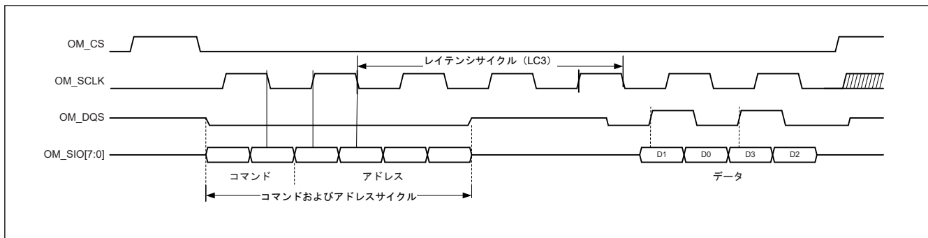
図 36.6 OctaRAM インタフェースでの書き込み動作の波形
