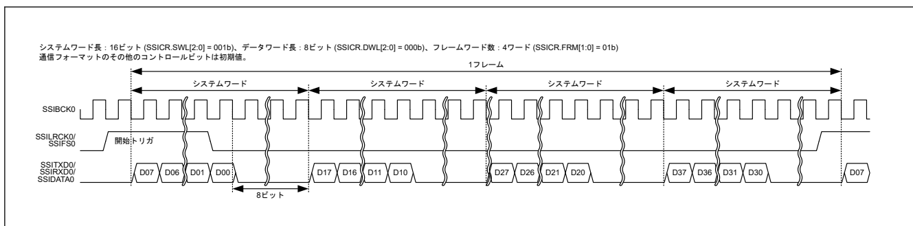
図 38.42 TDM フォーマット (パディングあり、システムワード長 > データワード長)
