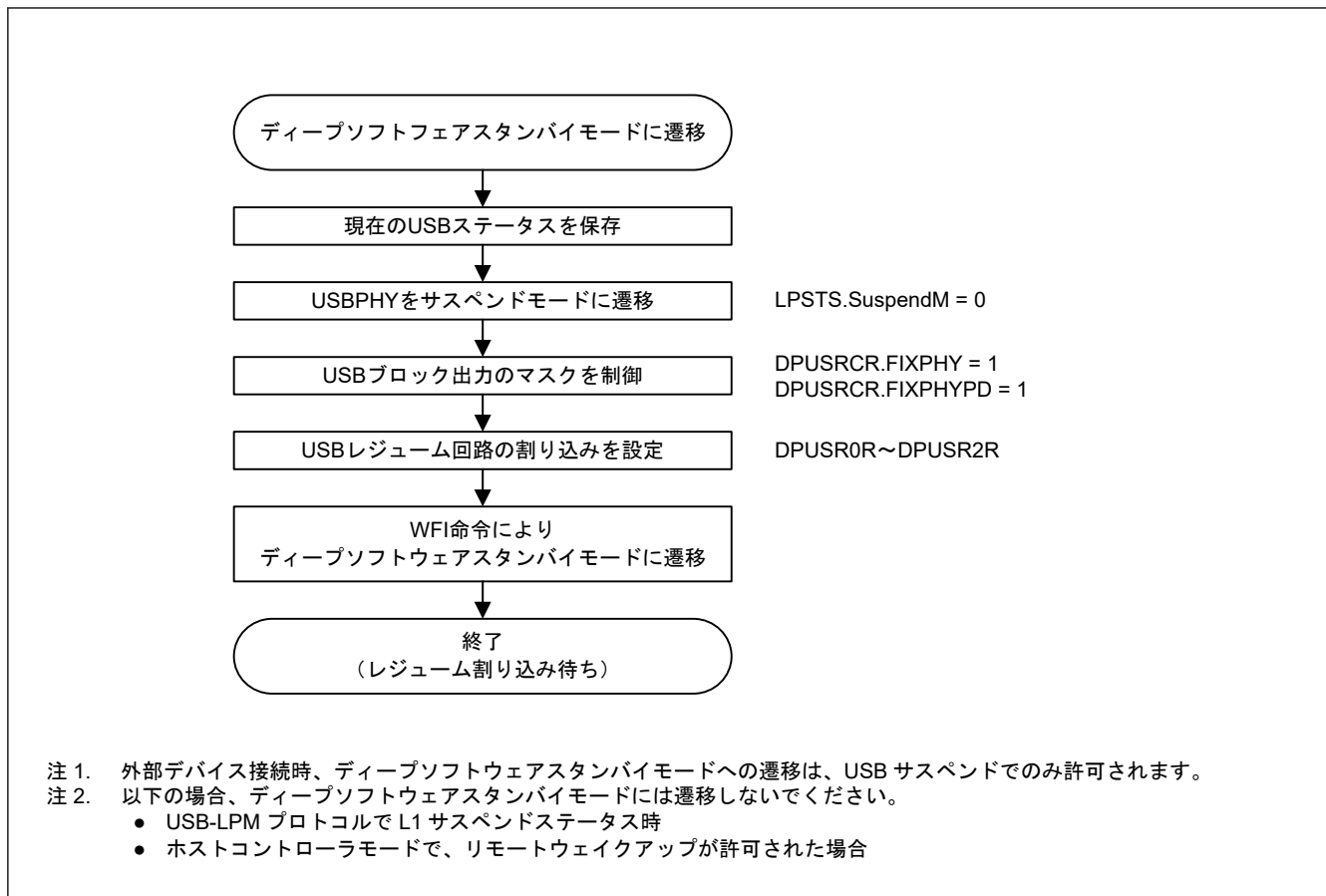
図 29.22 ホストコントローラまたはデバイスコントローラとしてディープソフトウェアスタンバイモードへ遷移する場合の USBHS 設定フロー
