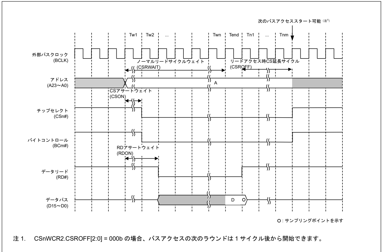
図 14.7 バスタイミング（ノーマルリード）（n = 0~7、m = 0~1）
