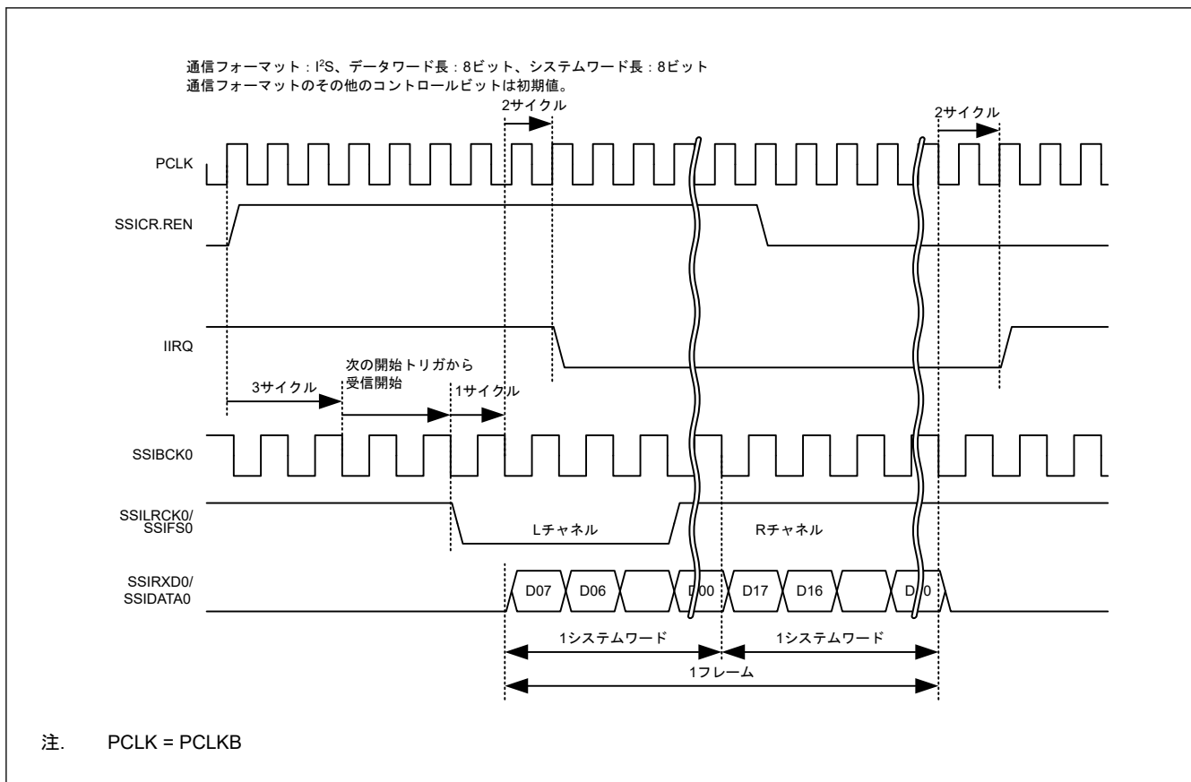
図 38.15 IIRQ 設定タイミング (受信)
