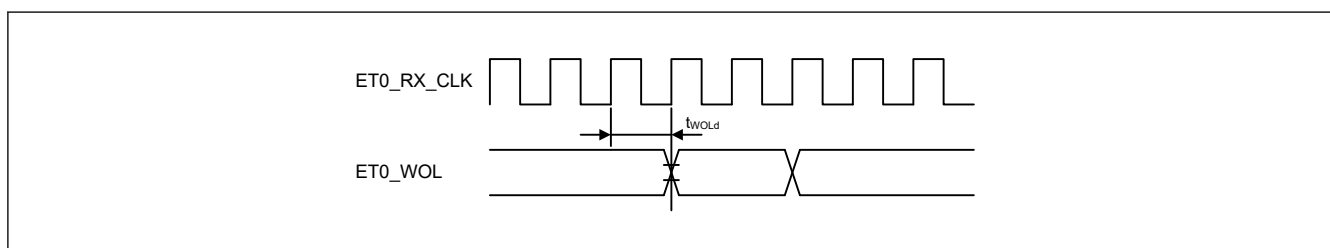
図 53.73 MII に対する WOL 出力タイミング
