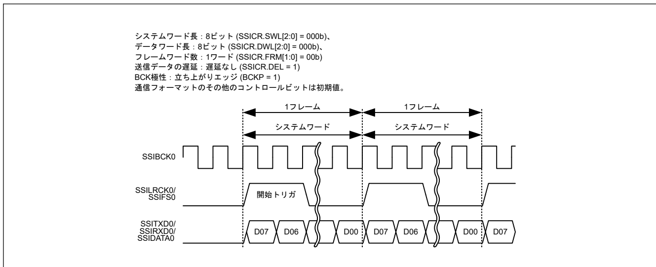
図 38.40 モノラルフォーマットにおけるロングフレーム (パディングなし)
