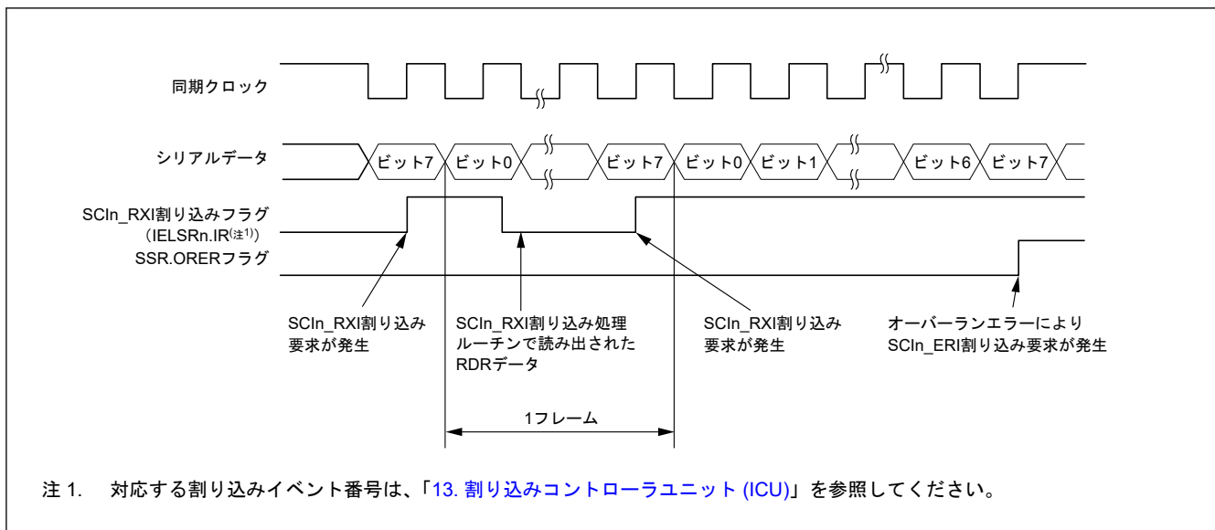
図 30.71 クロック同期式モードにおけるシリアル受信の動作例 (1) (RTS 機能を使用しない場合)
