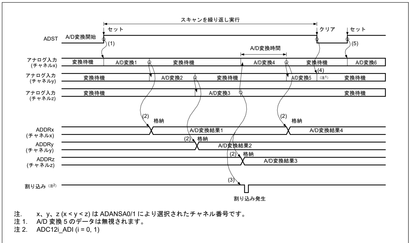
図 43.13 連続スキャンモードの基本動作例 (アナログ入力 (チャンネル x~z) 選択)
