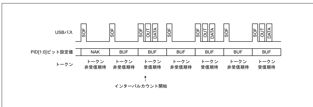
図 29.15 IITV[2:0] ≠ 0 の場合のフレームとトークン受信期待の関係
