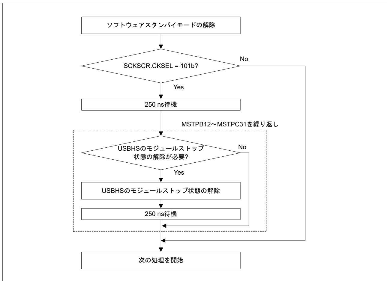
図 10.3 ソフトウェアスタンバイモード解除のフロー例
