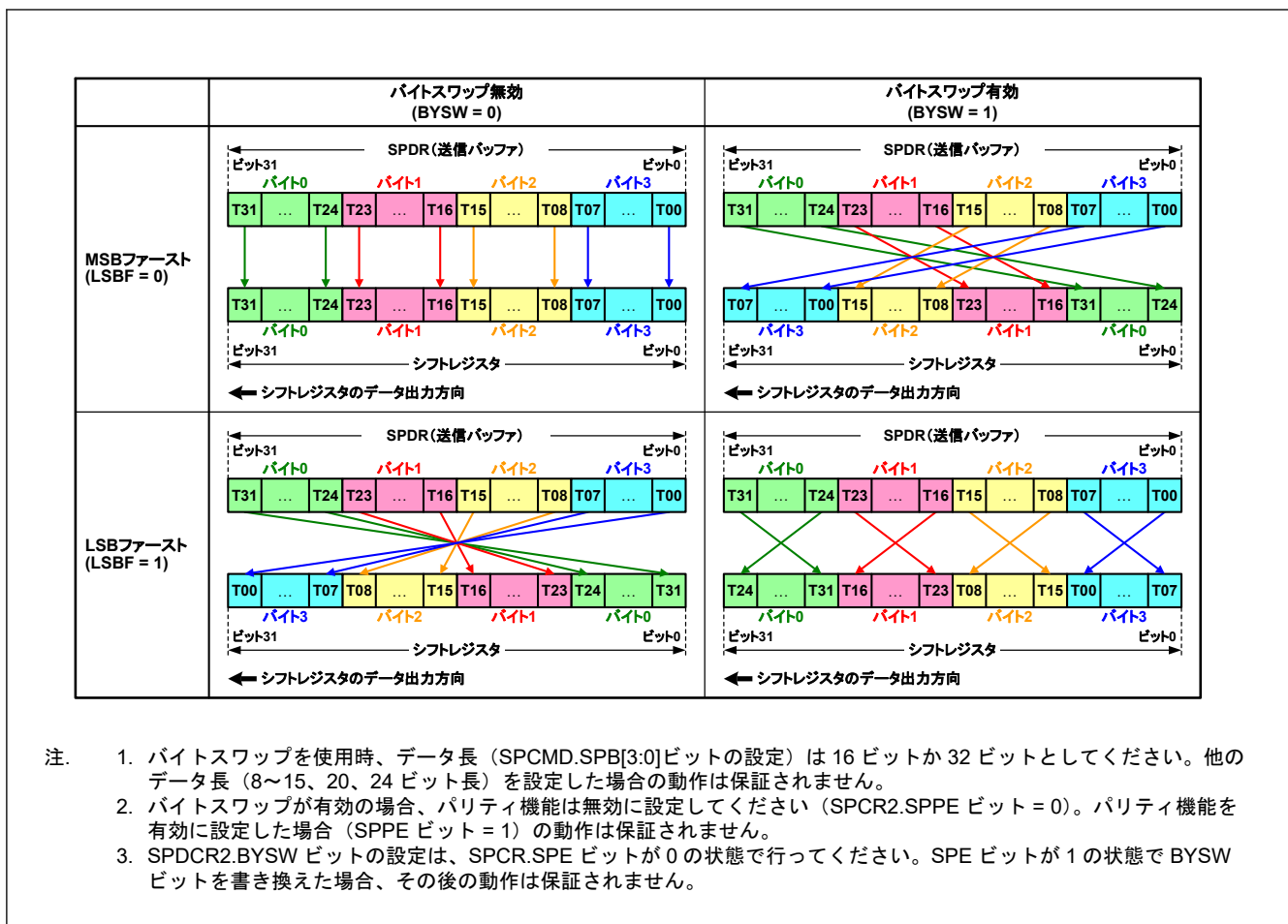
図 34.22 MSB/LSB 転送でのバイトスワップ
