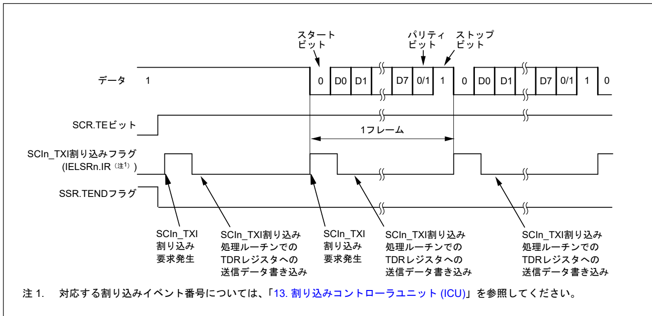
図 30.11 調歩同期式モードにおけるシリアル送信の動作例 (1) (8 ビットデータ/パリティあり/1ストップビット/CTS 機能不使用/送信開始時)
