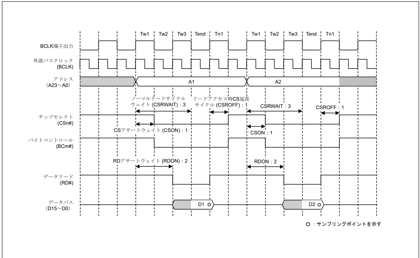
図 14.13 ノーマルリードアクセスの動作例 (EBCLK 端子出力選択ビットで BCLK の 2 分周を設定した場合) (n = 0~7、m = 0~1)
