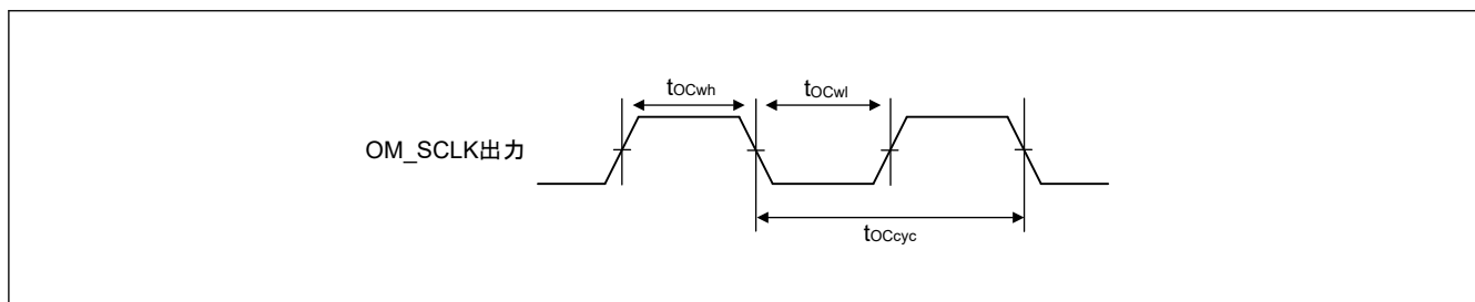
図 53.51 クロックタイミング
