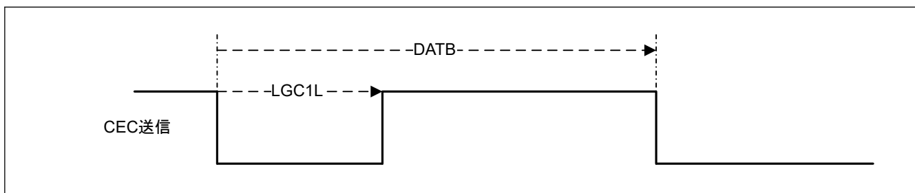
図 37.11 データビット (ロジカル 1) の出力波形
