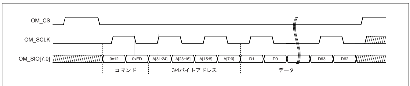
図 36.5 OctaFlash インタフェースでの書き込み動作の波形 (DOPI モード)
