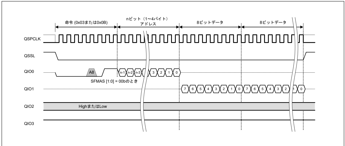
図 35.18 標準リードバスサイクル
