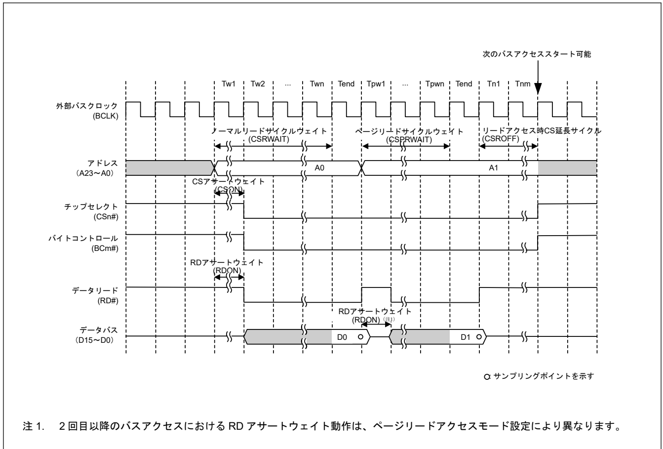
図 14.17 ページリードアクセスタイミング (n = 0~7、m = 0~1)
