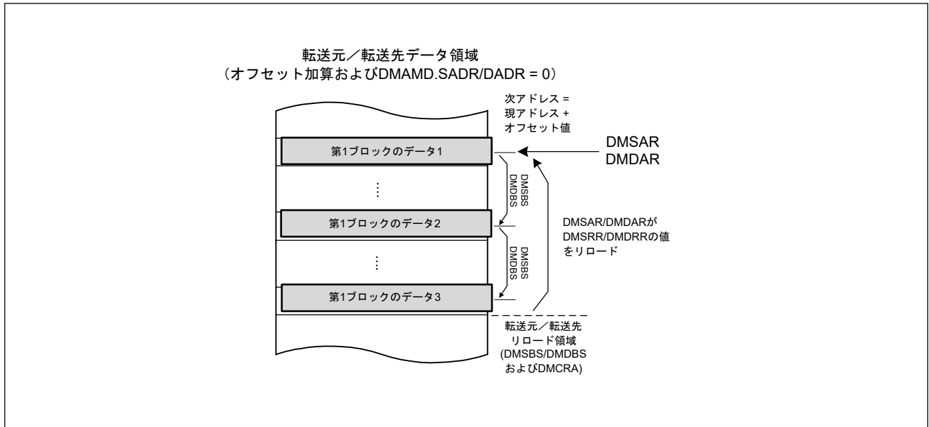
図 16.16 オフセット加算モードにおけるアドレス更新 (DMAMD.SADR = 0 かつ DMAMD.DADR = 0 の場合)
