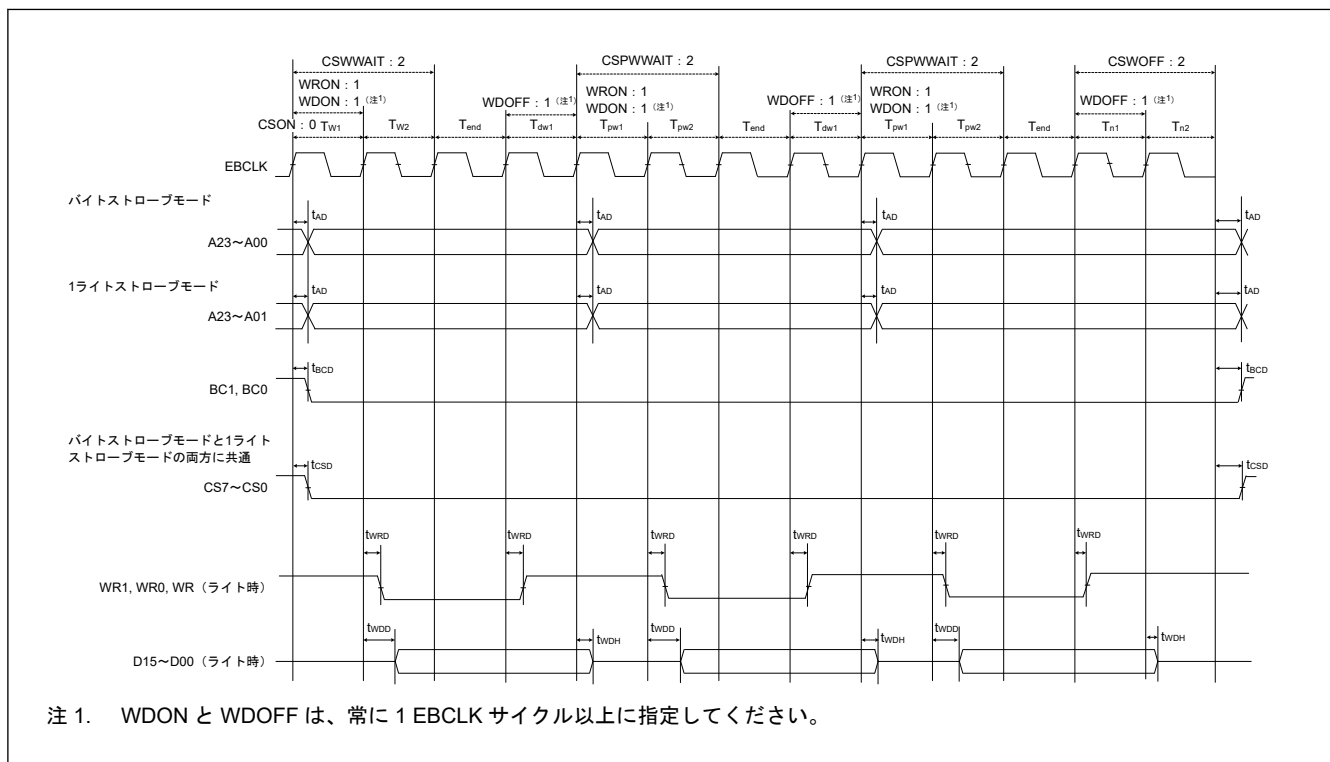
図 53.25 バスクロック同期を使用したページライトサイクルの外部バスタイミング
