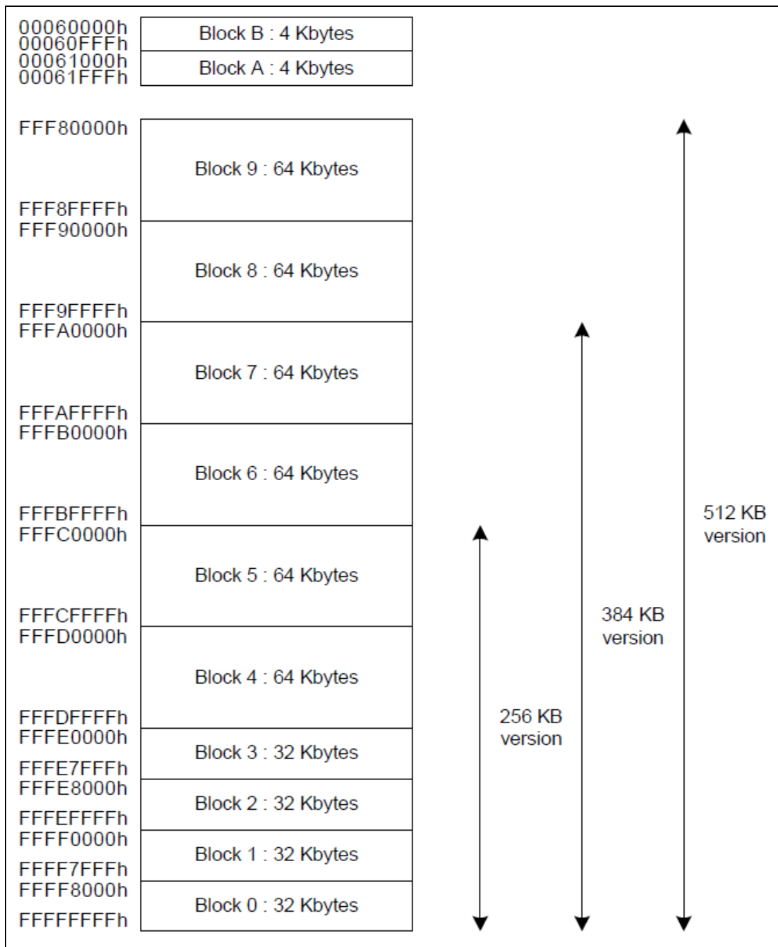
図 10-2: メモリマップ
