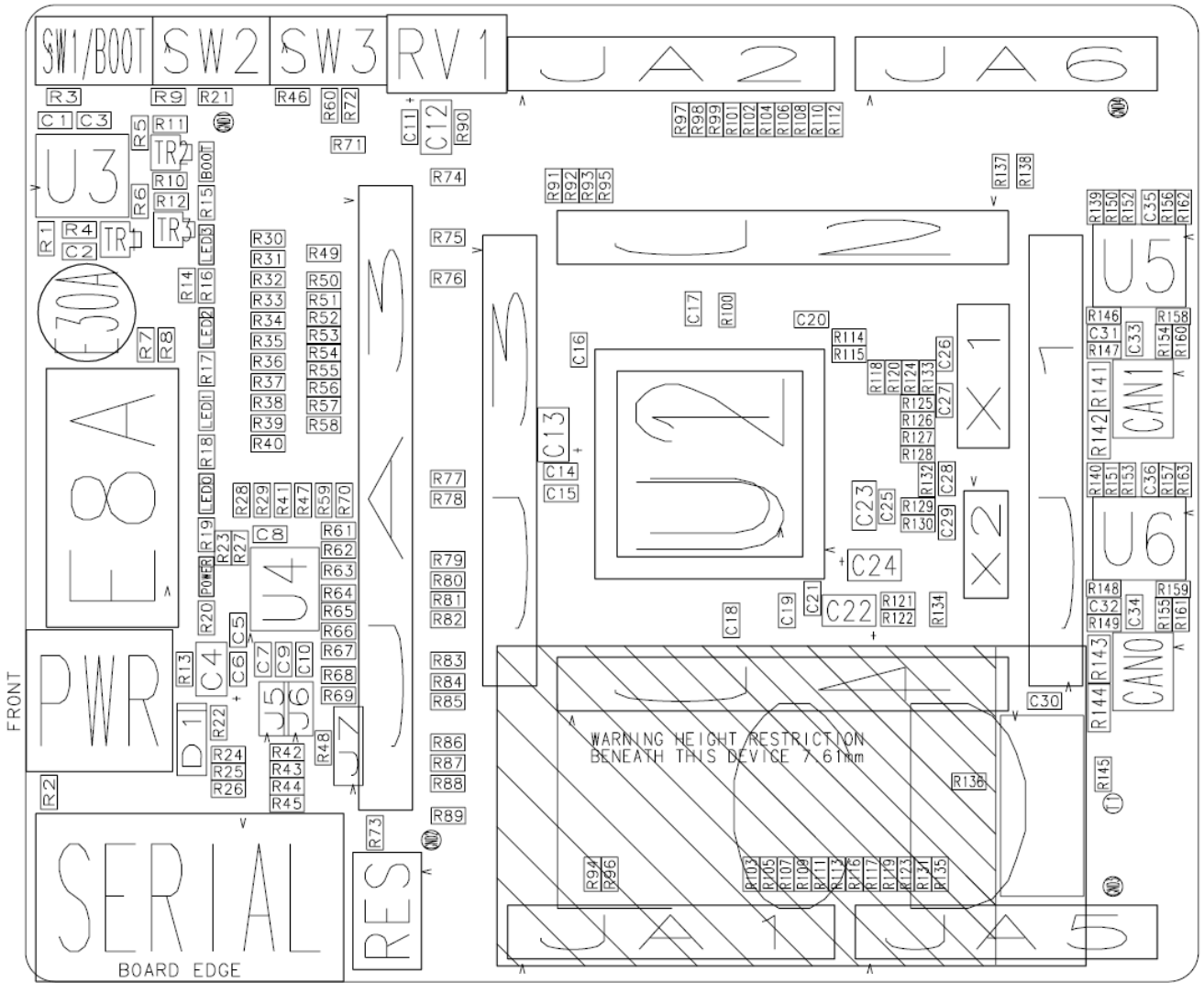
图 11-1: 部品配置图
