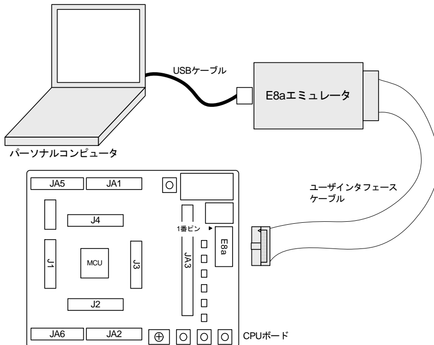
図 5-2: キット接続例
