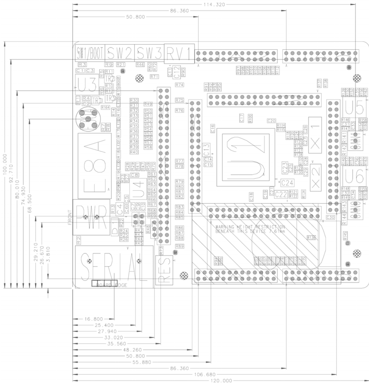
図 4-2: ボード寸法図
