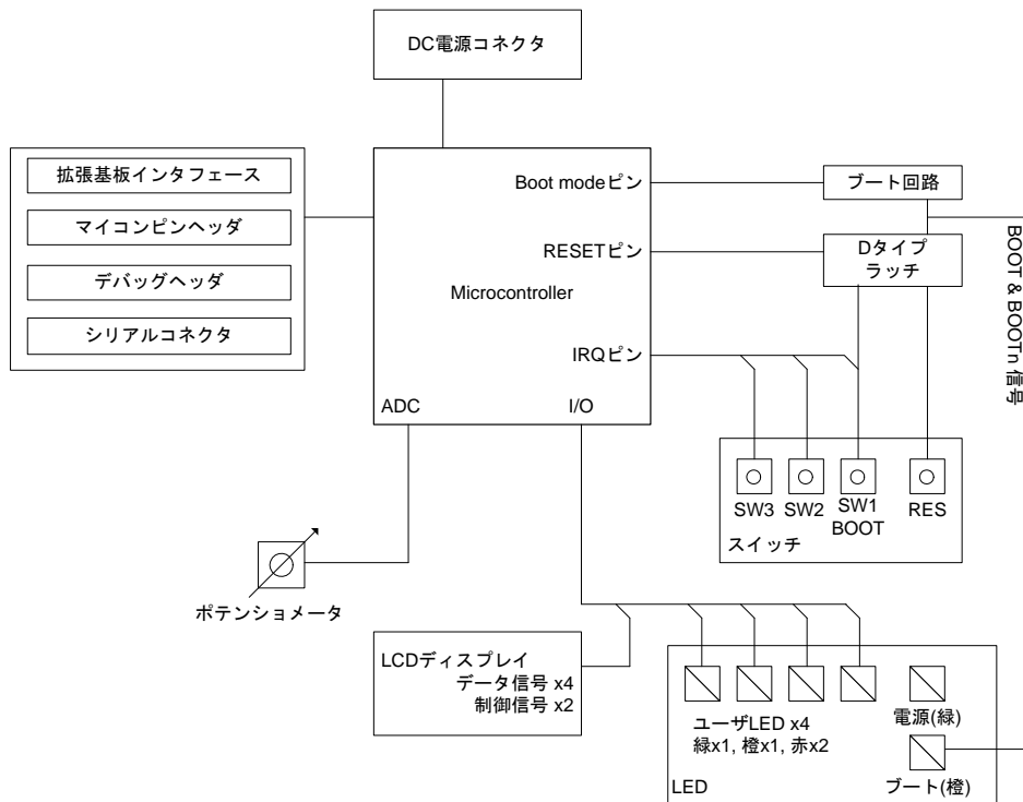
図 5-1: ブロック図
