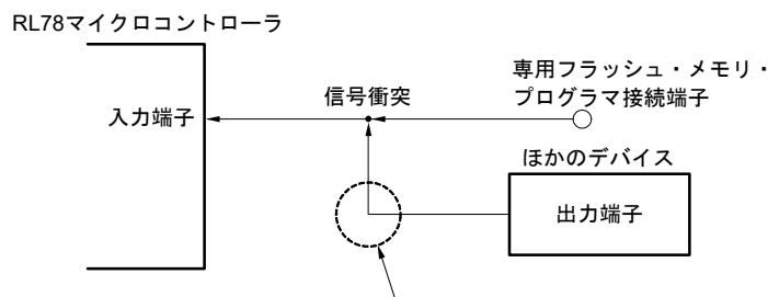
図25-5 信号の衝突 (RESET端子)
