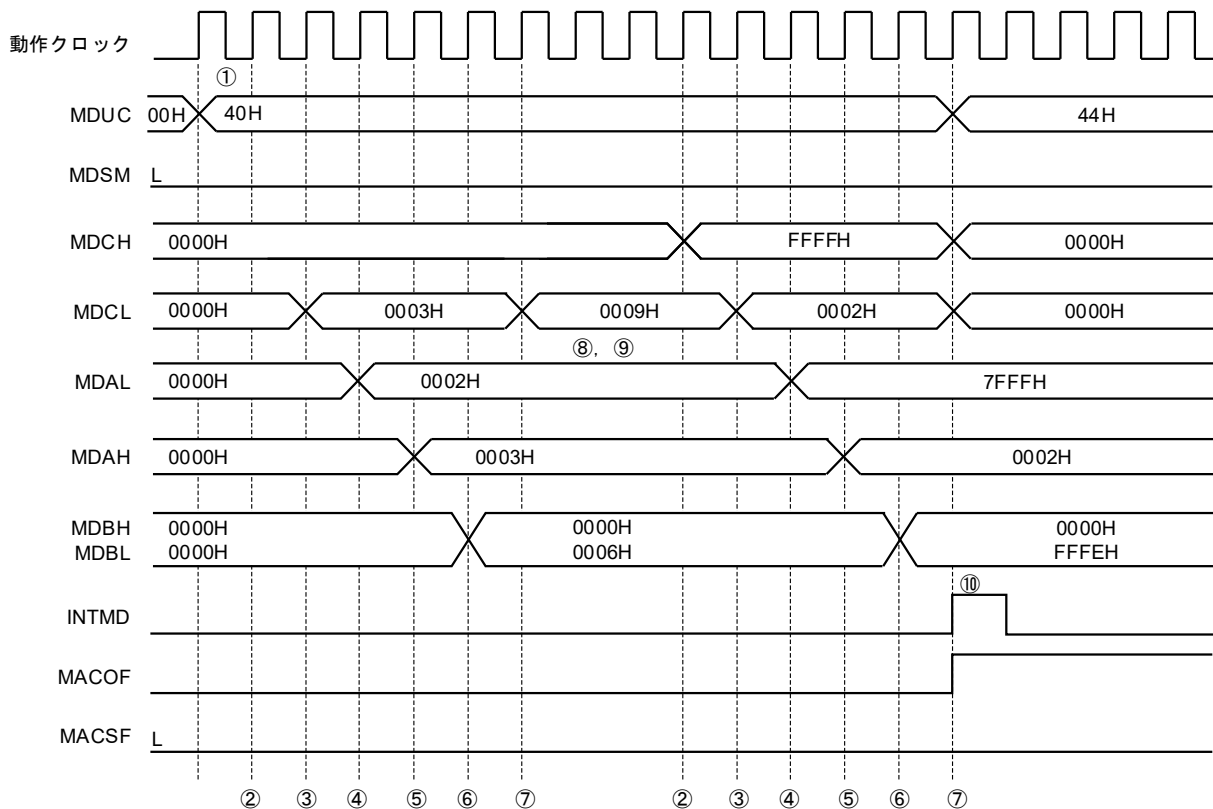
図14-8 積和演算（符号なし）動作のタイミング図 (2×3+3=9 → 32767×2+4294901762=0 (オーバーフロー発生))
