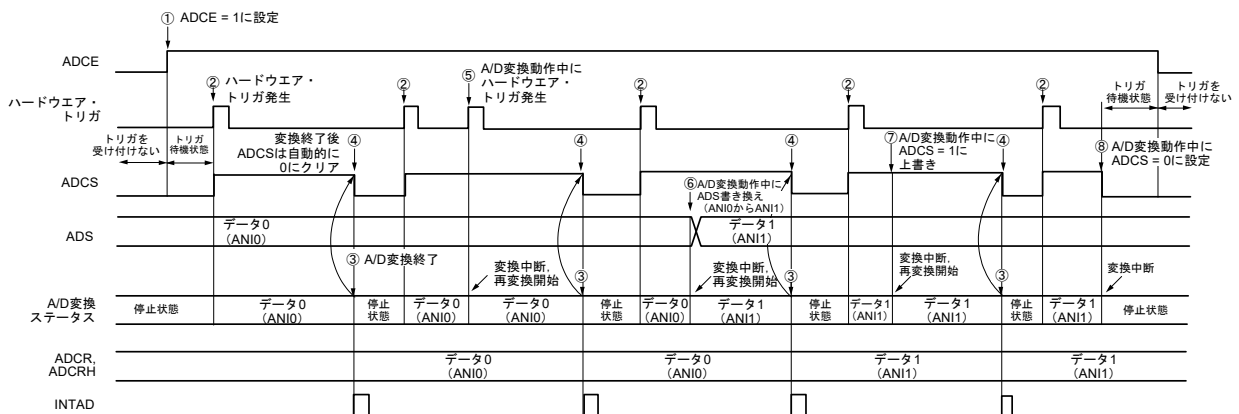
図11-26 ハードウェア・トリガ・ウエイト・モード (セレクト・モード, ワンショット変換モード) 動作タイミング例
