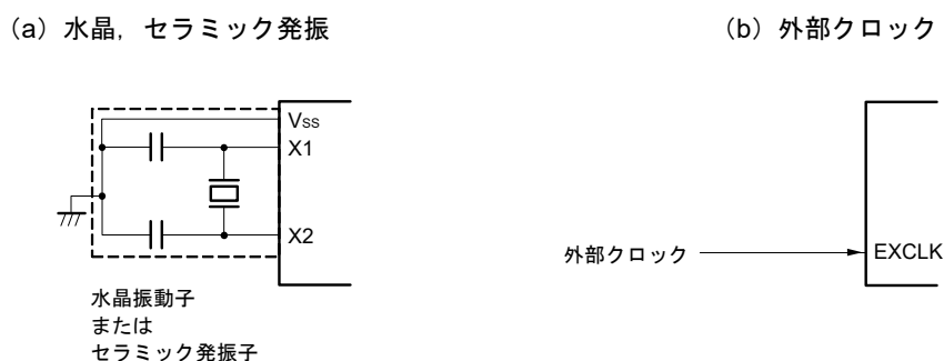
図5-11 X1発振回路の外付け回路例
