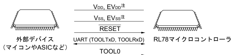
図25-3 フラッシュ・メモリにプログラムを書き込むための環境
