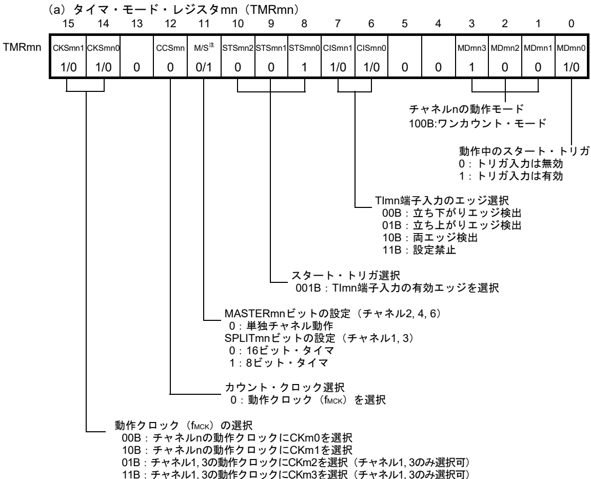
図6-63 デイレイ・カウンタ機能時のレジスタ設定内容例
