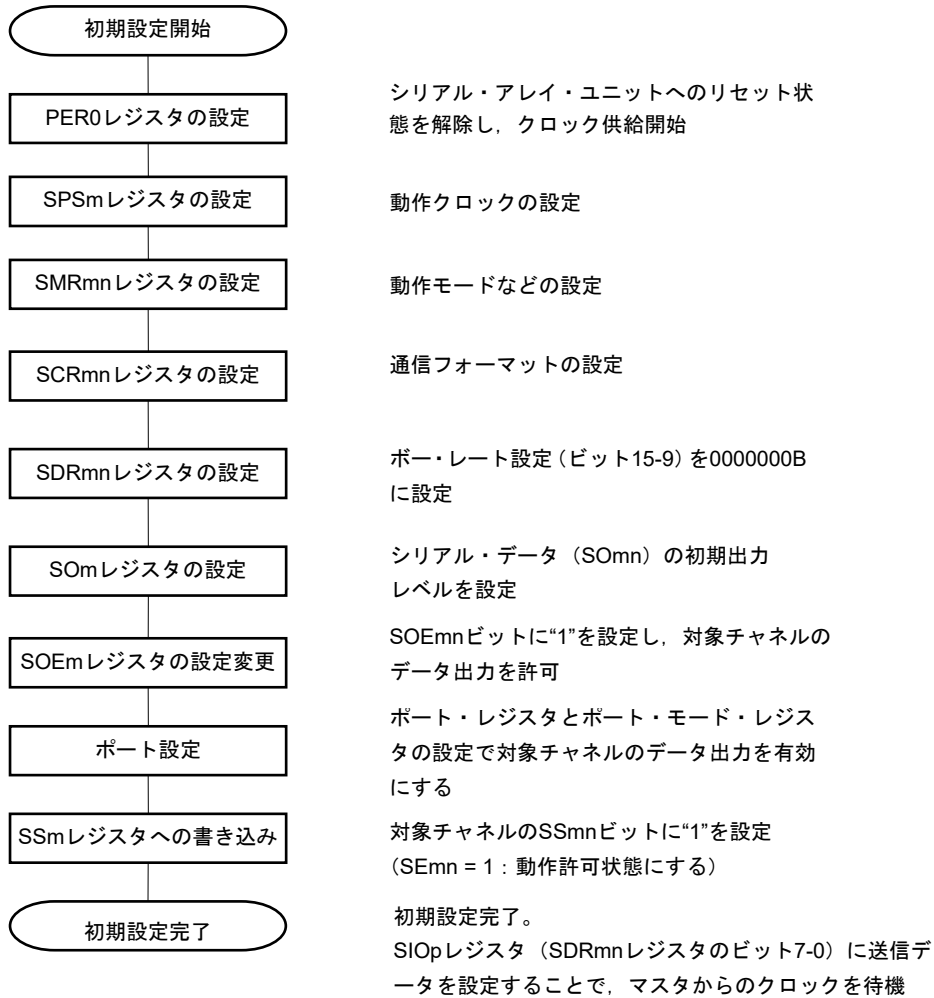
図12-64 スレーブ送受信の初期設定手順
