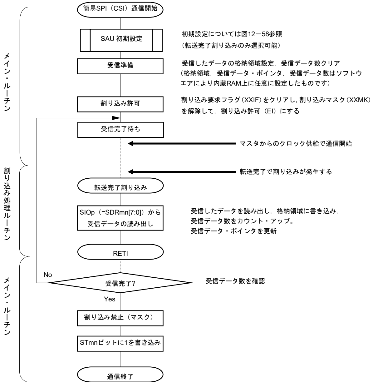
図12-62 スレーブ受信（シングル受信モード時）のフロー・チャート
