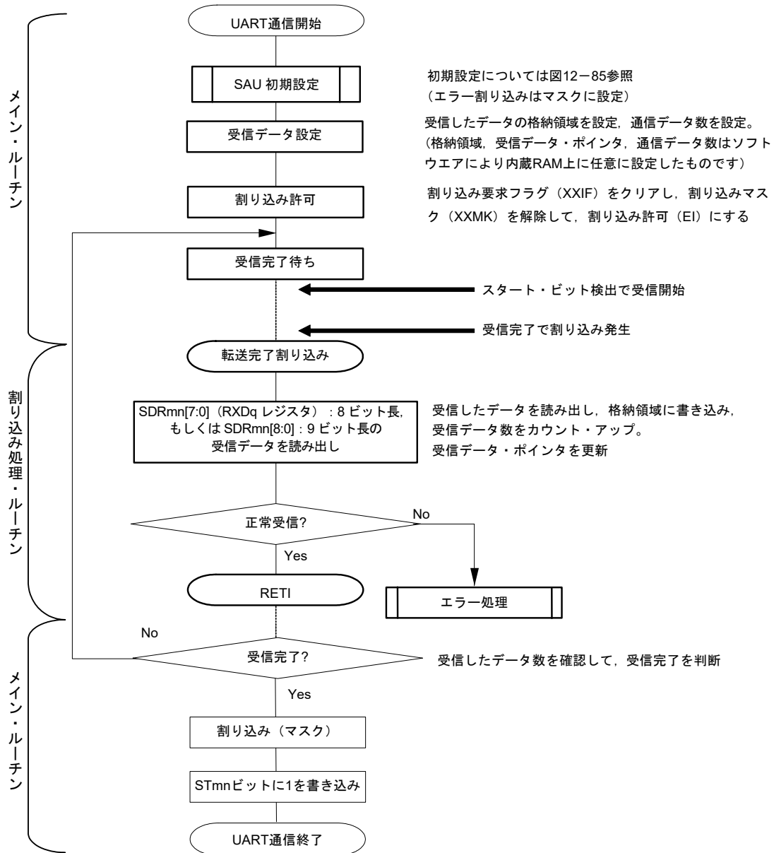
図12-89 UART受信のフロー・チャート
