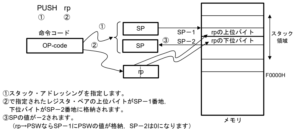
図3-41 PUSH rpの例
