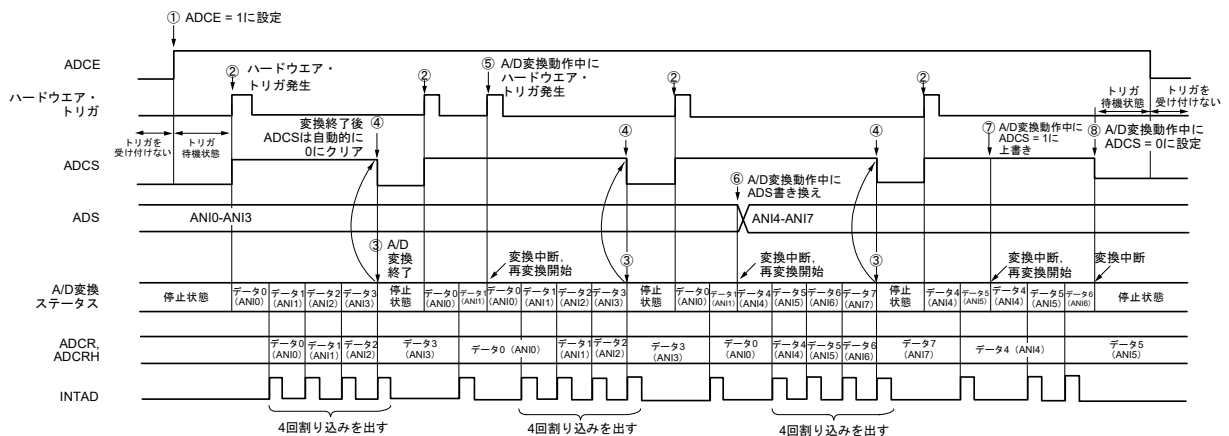
図11-28 ハードウェア・トリガ・ウエイト・モード（スキャン・モード，ワンショット変換モード） 動作タイミング例
