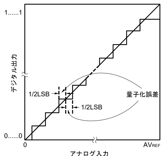
図11-39 量子化誤差
