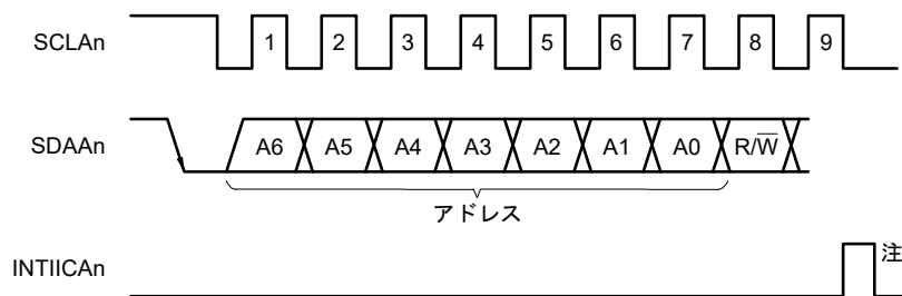
図13-16 アドレス
