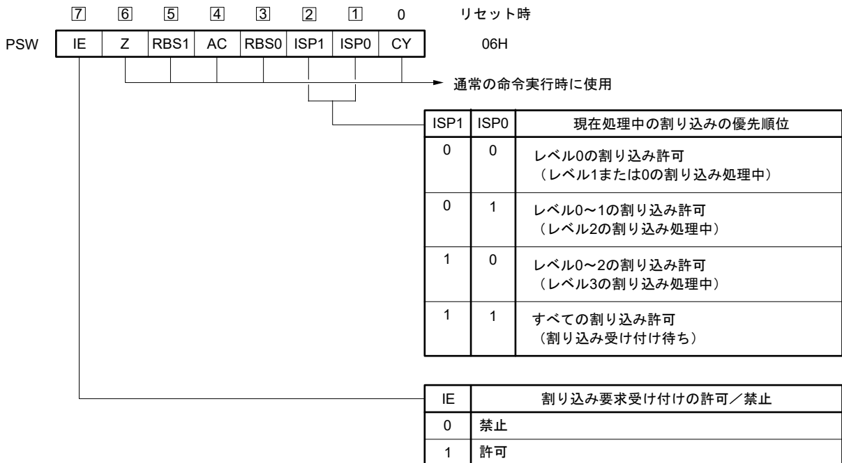
図16-6 プログラム・ステータス・ワードの構成
