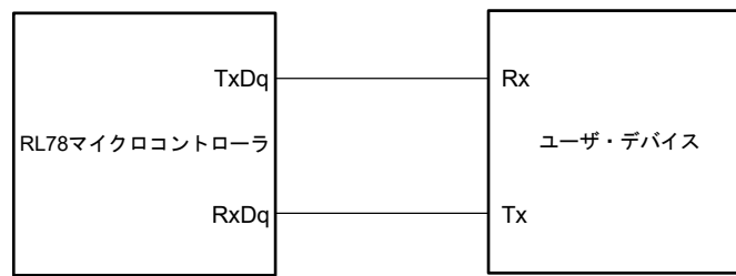
UARTモード接続図 (同電位通信時)
