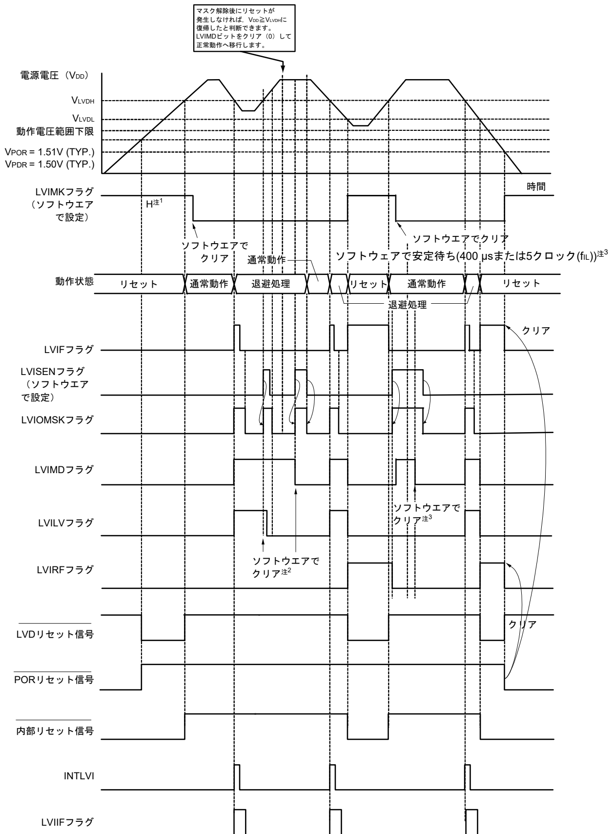
図21-7 割り込み&リセット信号発生タイミング (オプション・バイトのLVIMDS1, LVIMDS0 = 1, 0) (1/2)
