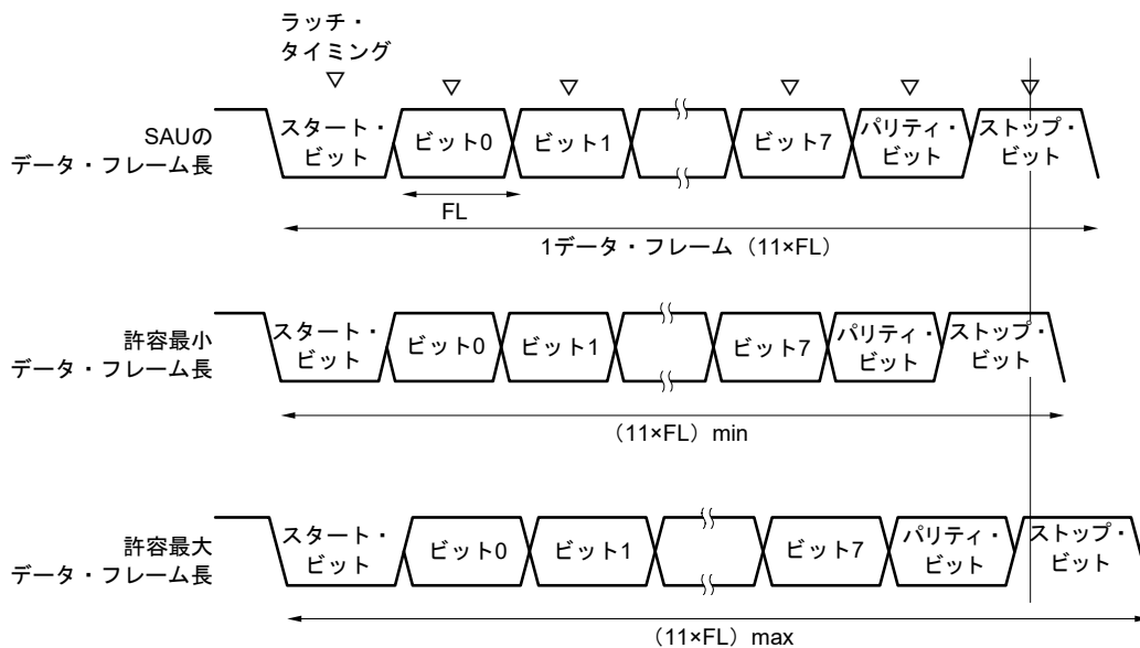
図12-95 受信時の許容ポー・レート範囲 (1データ・フレーム長 = 11ビットの場合)
