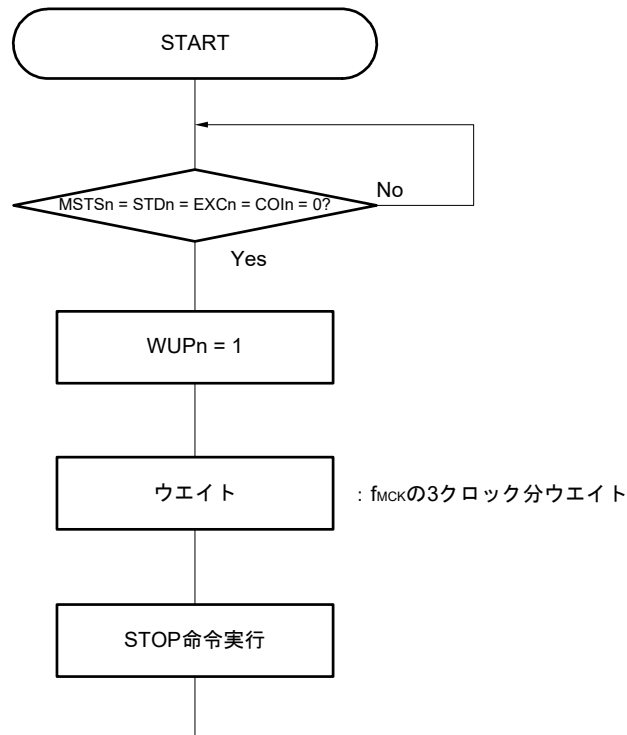
図13-22 WUPn = 1を設定する場合のフロー
