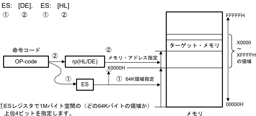
図3-31 ES:[DE], ES:[HL]の例
