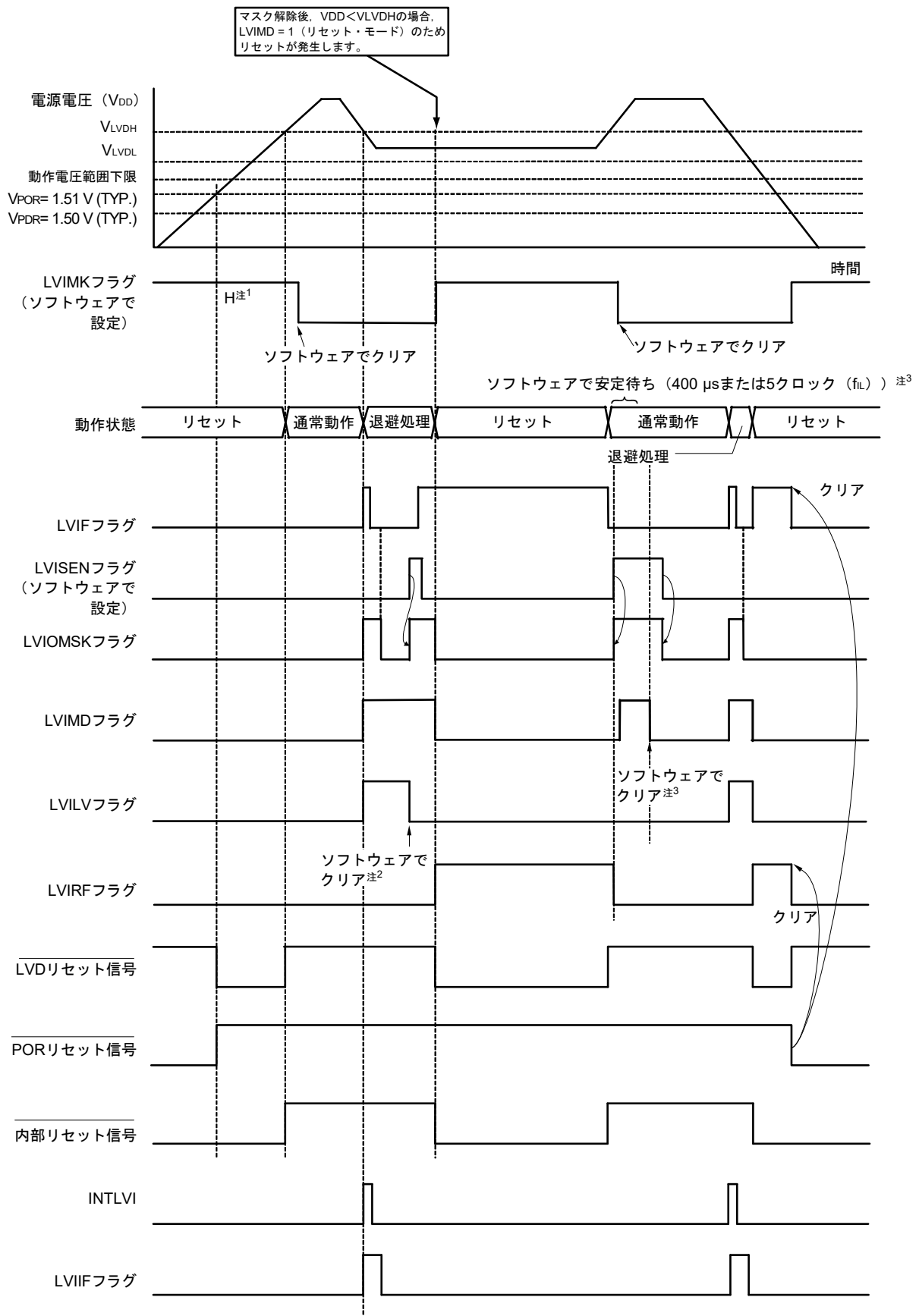
図21-7 割り込み&リセット信号発生タイミング (オプション・バイトのLVIMDS1, LVIMDS0 = 1, 0) (2/2)
