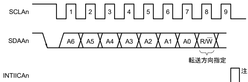
図13-17 転送方向指定
