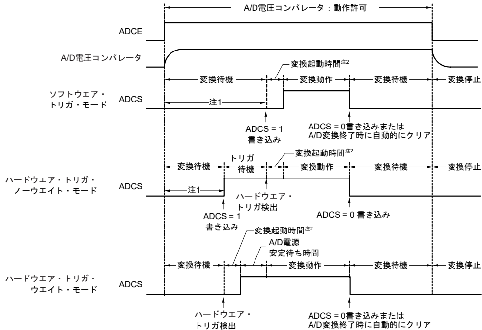
図11-4 A/D電圧コンパレータ使用時のタイミング・チャート
