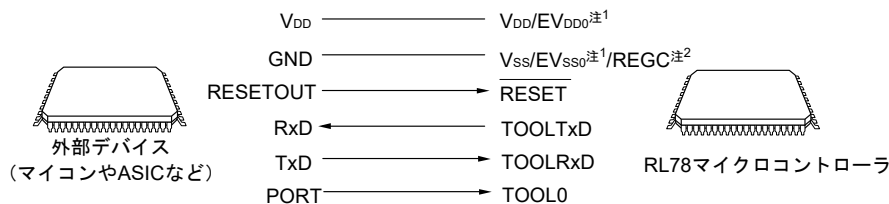
図25-4 外部デバイスとの通信
