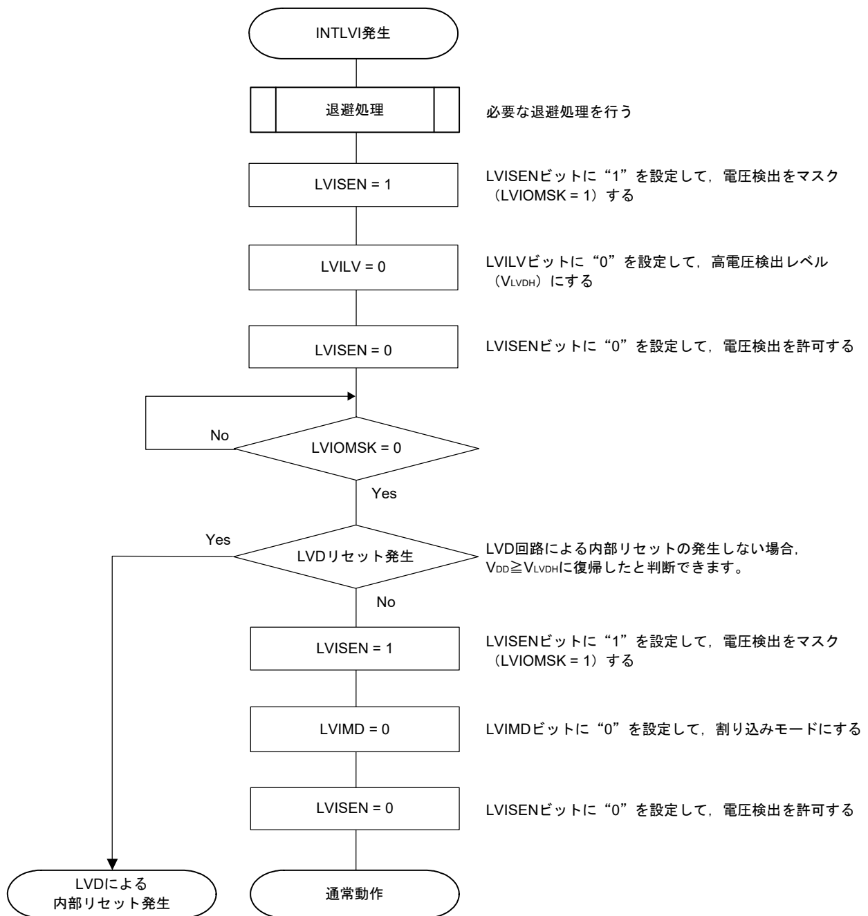
図21-8 動作電圧確認／リセットの設定手順
