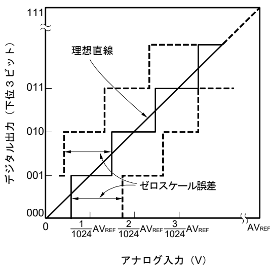
図11-40 ゼロスケール誤差
