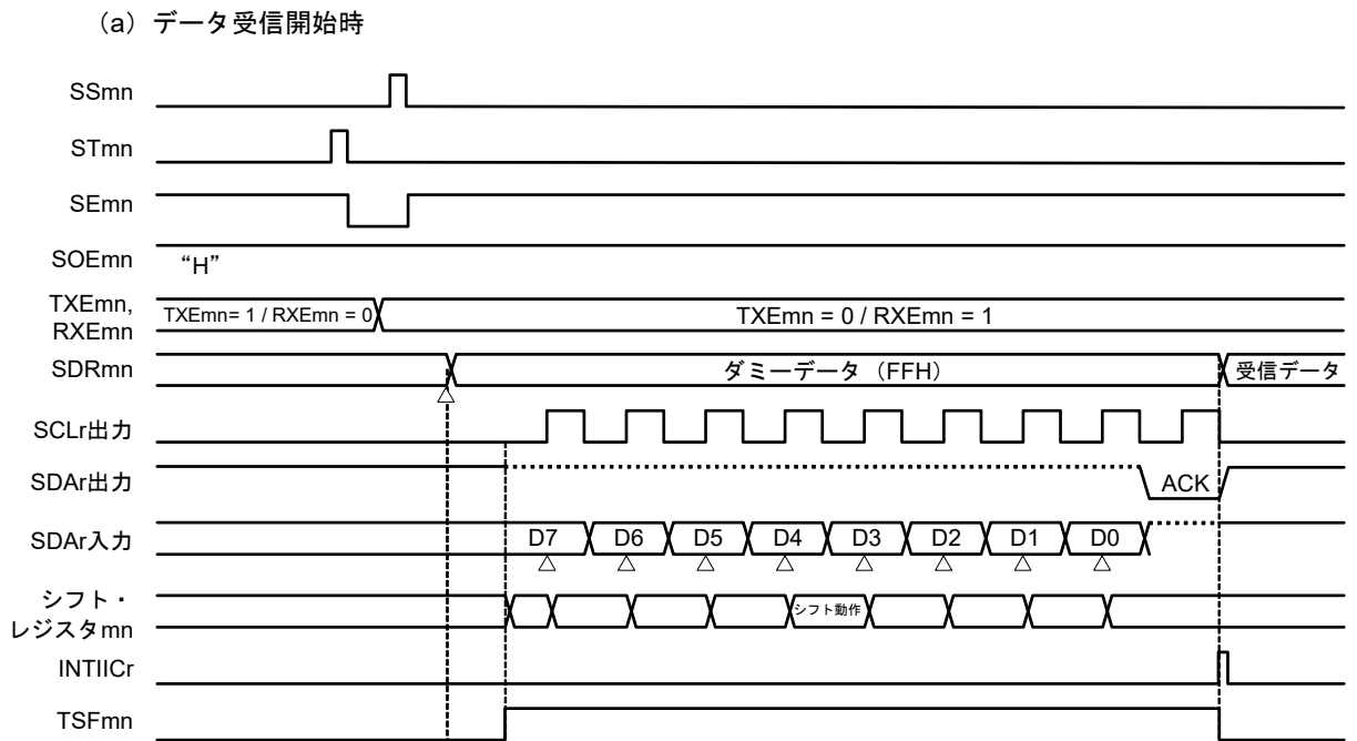
図12-112 データ受信のタイミング・チャート
