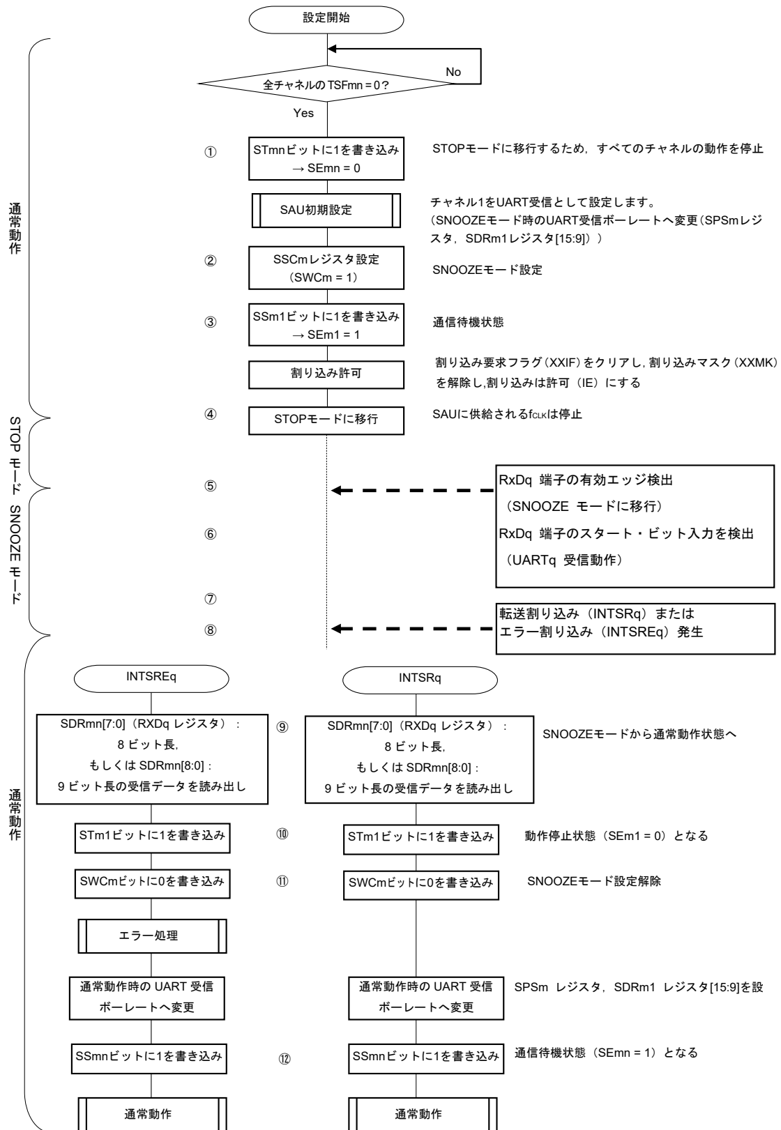
図12-92 SNOOZEモード動作 (EOCm1 = 0, SSECm = 0/1もしくはEOCm1 = 1, SSECm = 0) 時の フロー・チャート
