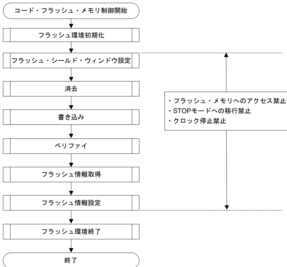
図25-8 セルフ・プログラミング（フラッシュ・メモリの書き換え）の流れ
