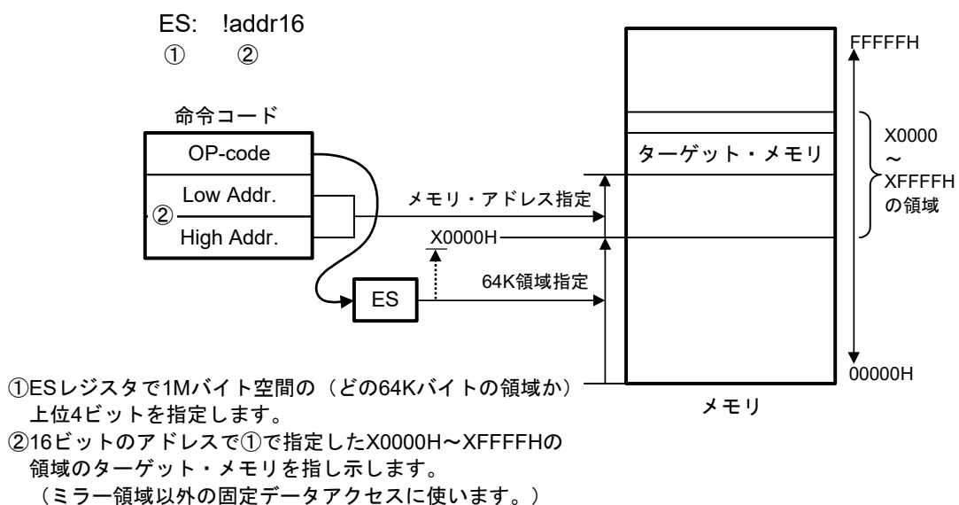
図3-27 ES:!addr16の例
