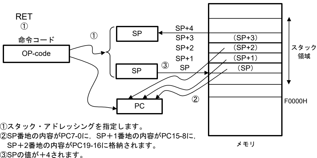
図3-44 RETの例
