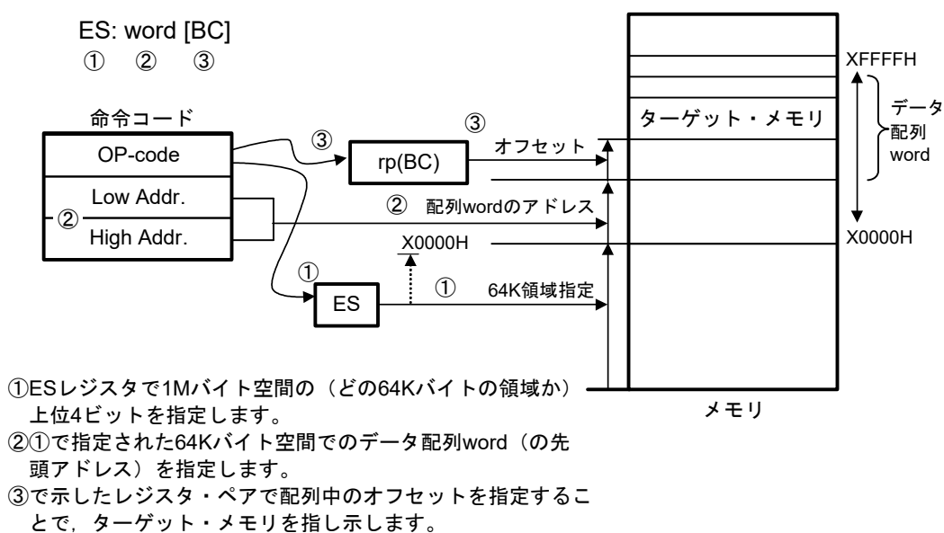
図3-38 ES:word[BC]の例
