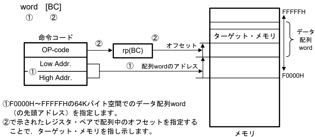
図3-35 word[BC]の例
