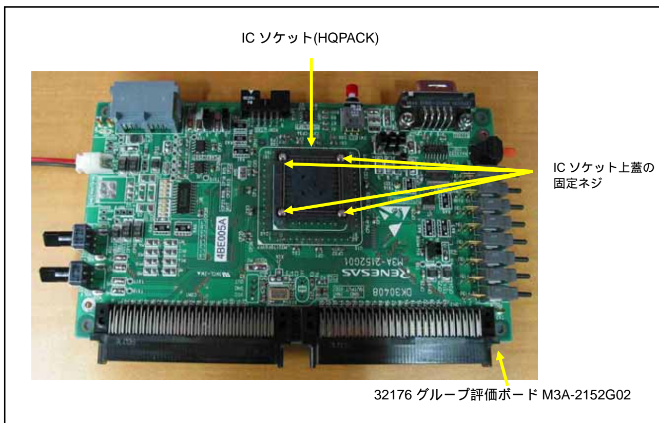
図 3.2 評価ボード M3A-2152G02 の例
