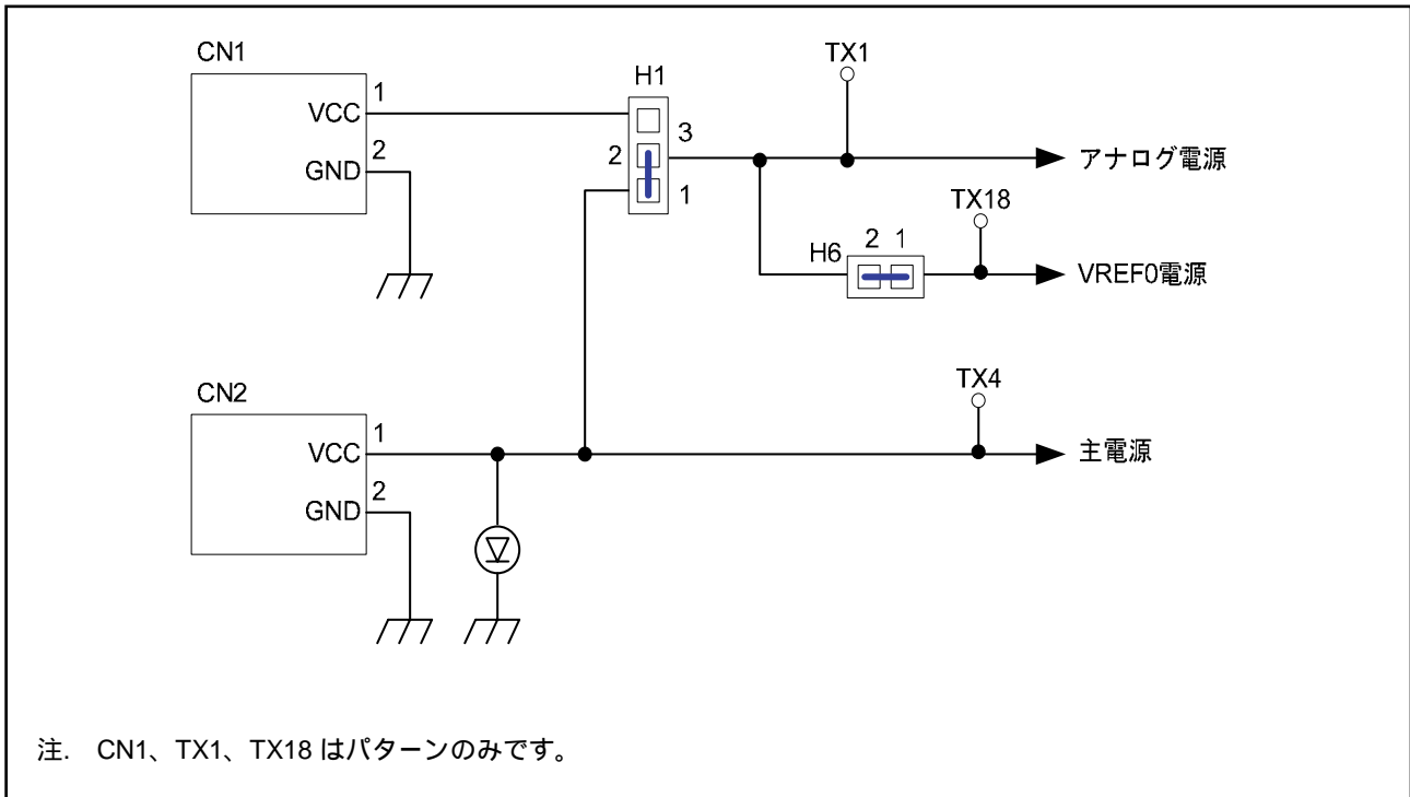
図 2.1 電源供給回路
