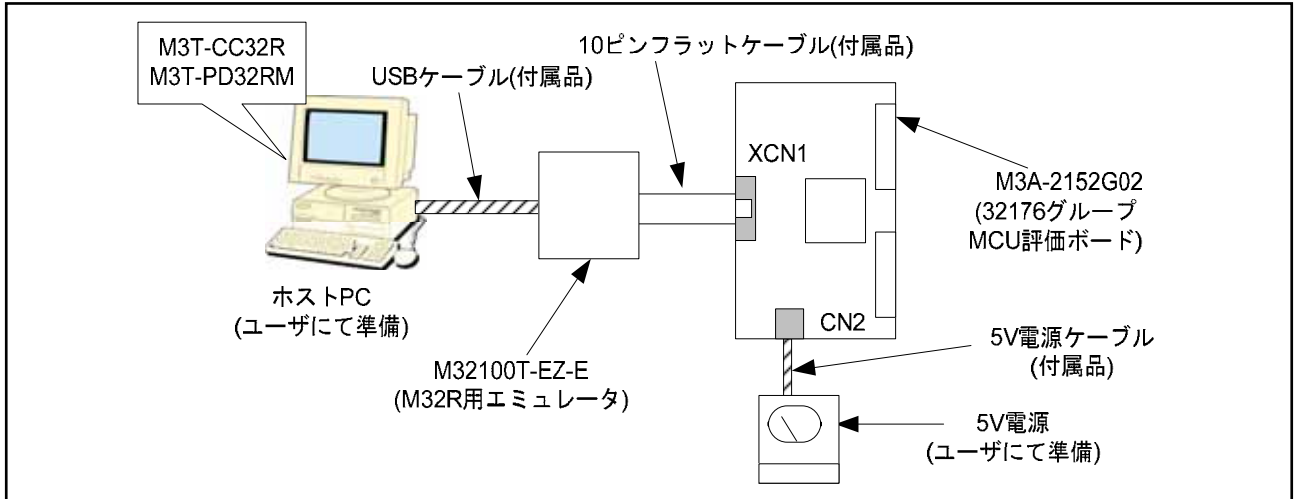
図 1.1 付属エミュレータ接続時の M3A-2152G52A システム構成例
