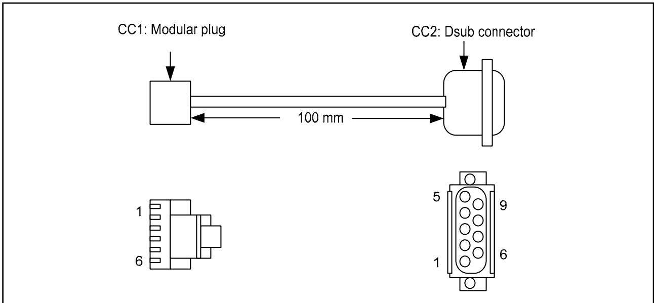
図 3.3 外観
