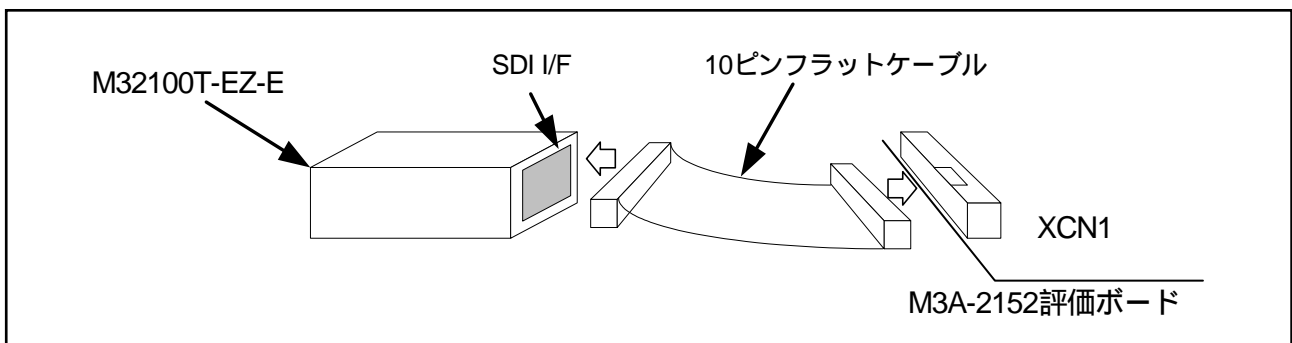
図 5.3 M3A-2152 評価ボードと M32100T-EZ-E の接続
