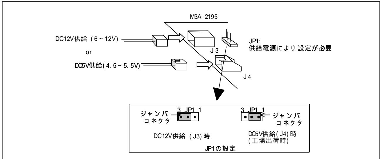
図 5.4 M3A-2195 電源供給時の接続
