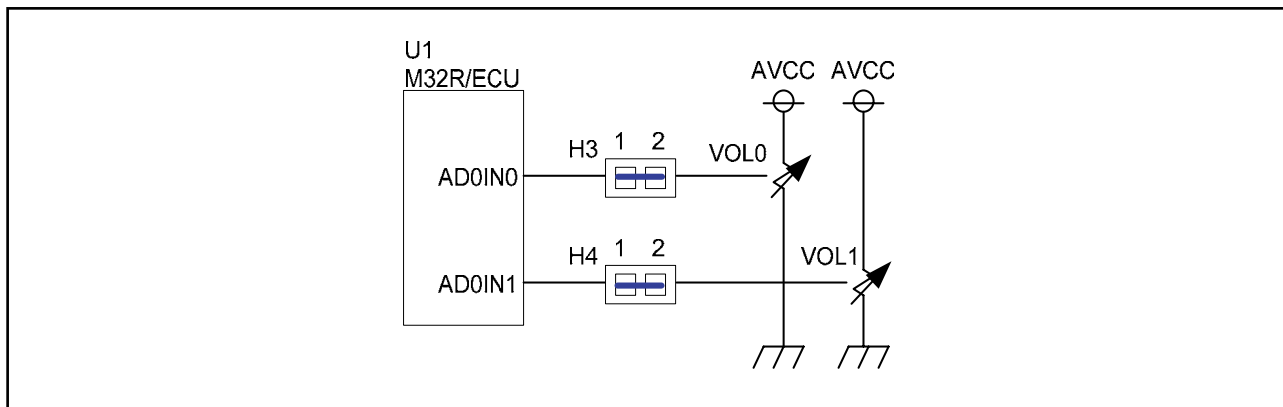
図 2.9 アナログポート入力制御回路
