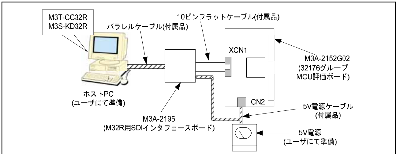
図 1.2 付属エミュレータ接続時の M3A-2152G52 用システム構成例
