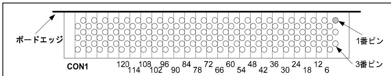
図 3.1 部品実装面側から見た CON1 拡張コネクタピン配置図
