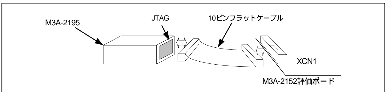
図 5.7 M3A-2152 評価ボードと M3A-2195 の接続
