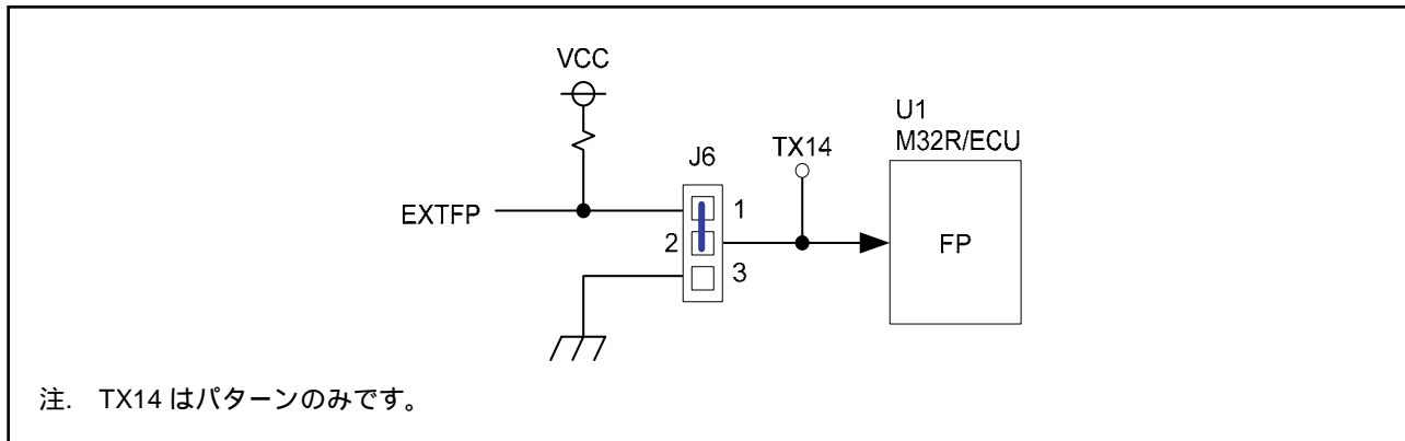
図 2.2 FP 選択回路
