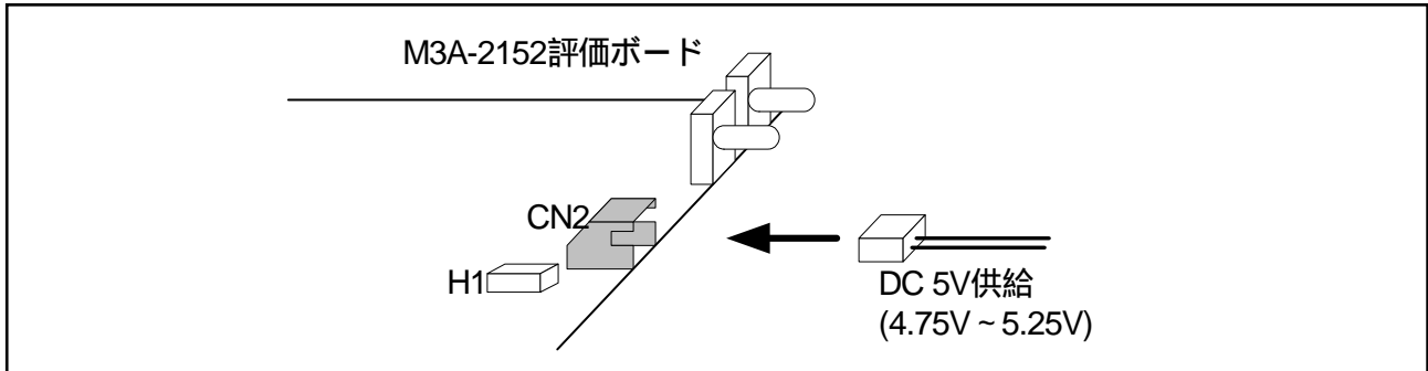
図 5.6 M3A-2152 評価ボード電源供給時の接続
