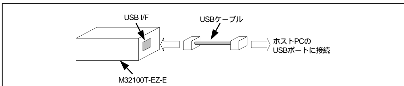
図 5.1 M32100T-EZ-E とホスト PC の接続
