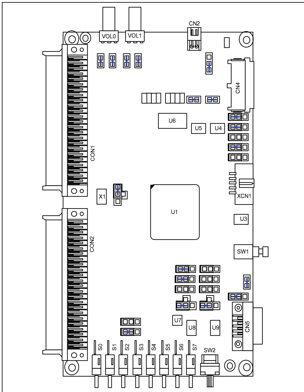
図 1.2 外観図
