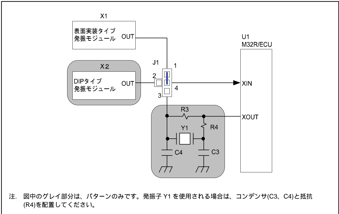
図 2.5 発振回路
