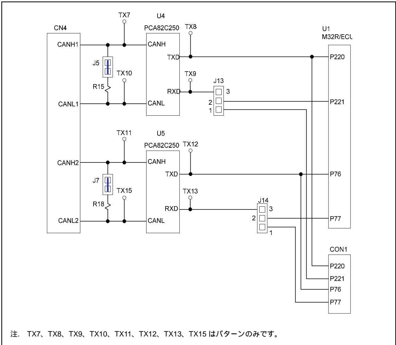
図 2.10 CAN 搭載システムとのインタフェース
