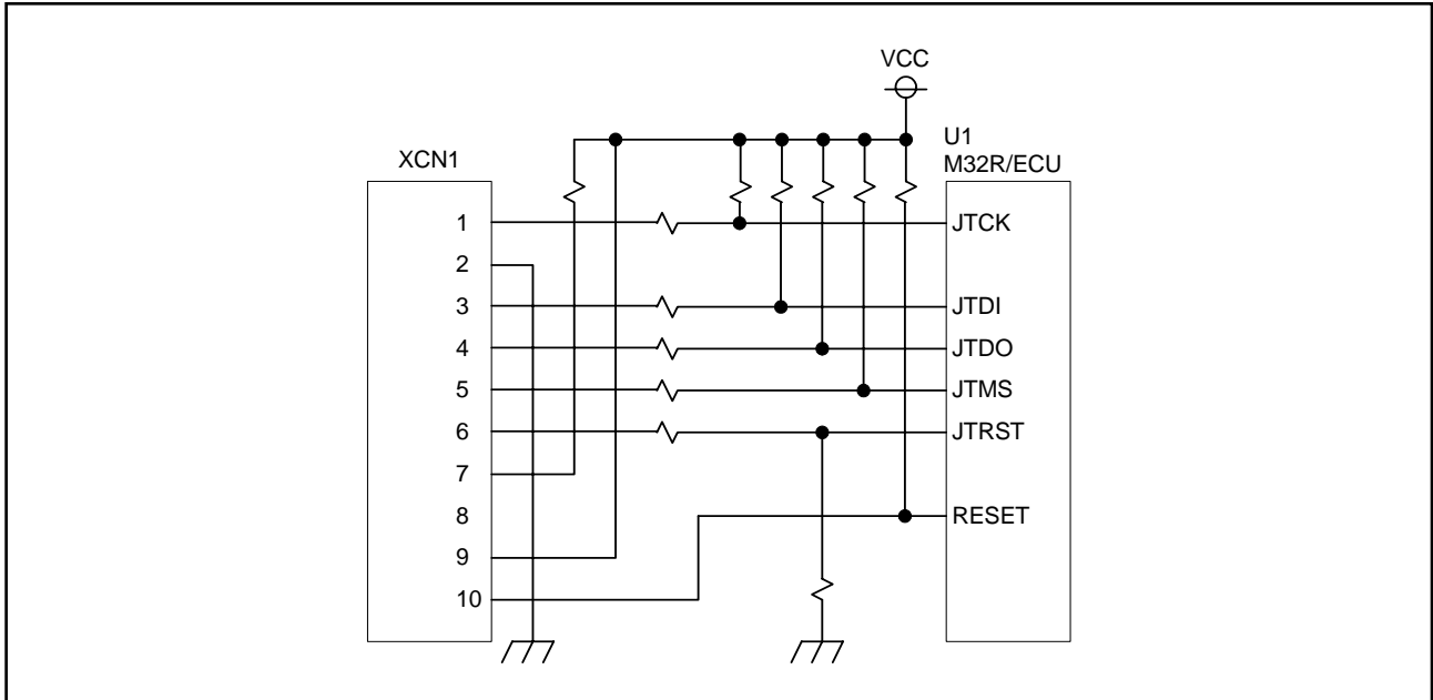
図 2.11 JTAG 周辺回路
