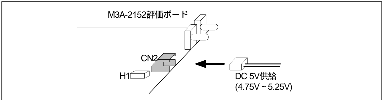
図 5.8 M3A-2152 評価ボード電源供給時の接続
