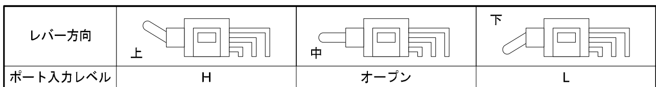
図 2.8 トグルスイッチのポジション
