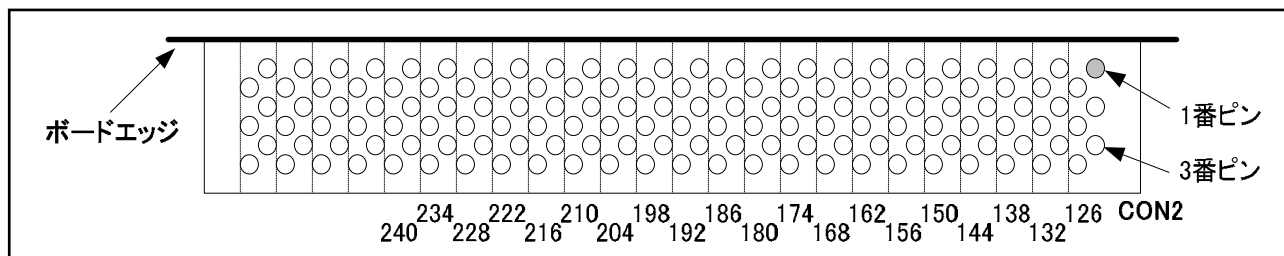
図 3.2 部品実装面側から見た CON2 拡張コネクタピン配置図
