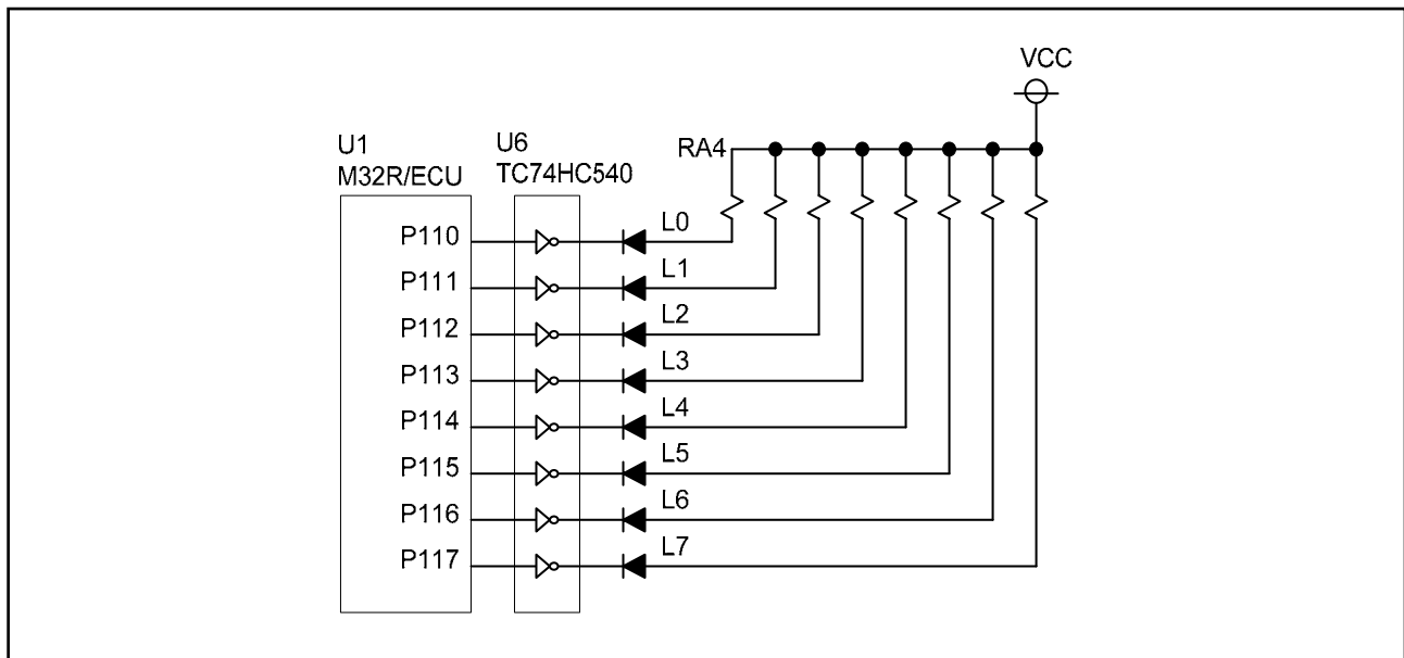
図 2.6 汎用出力ポートの LED 表示ブロック
