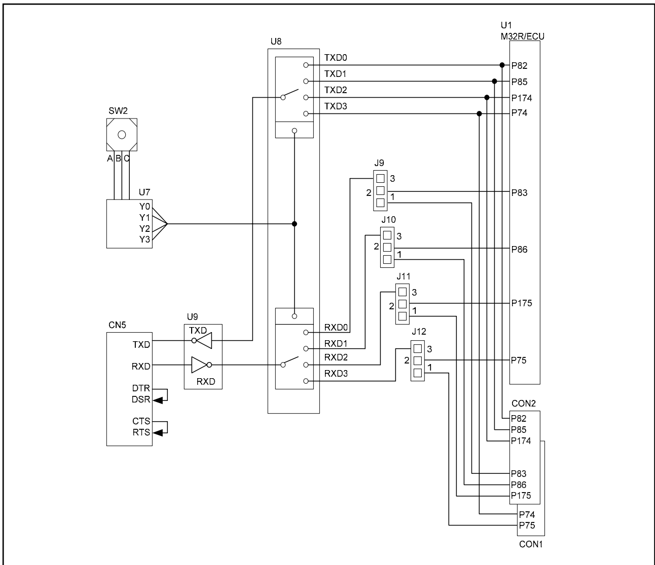
図 2.4 シリアル I/O インタフェース
