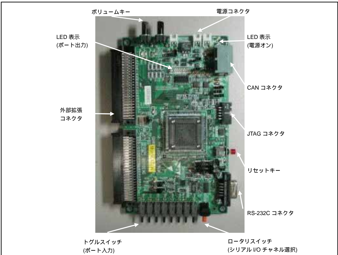
図 1.1 評価ボード写真
