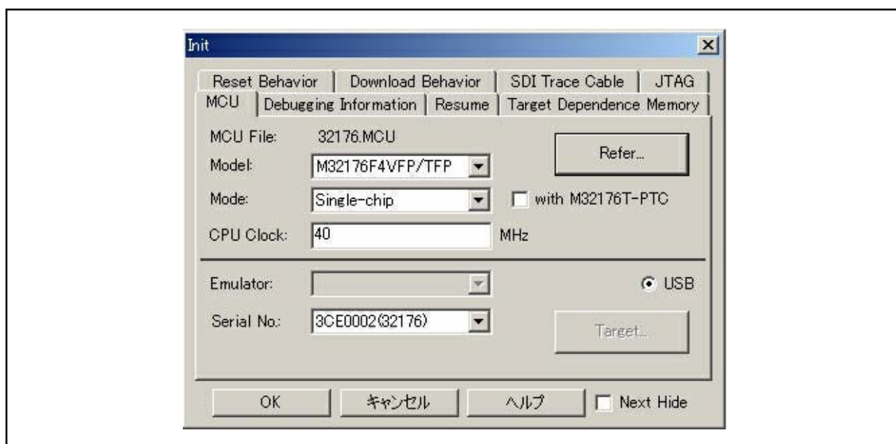
図 6.2 M3T-PD32RM 初期設定ダイアログ
