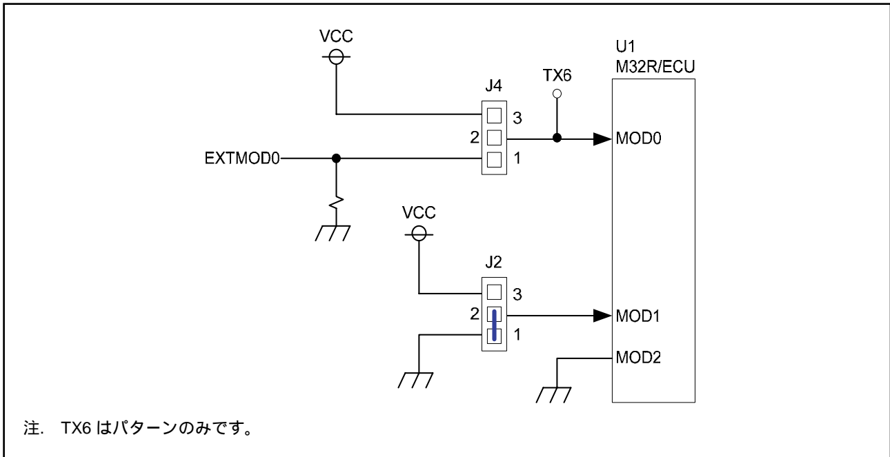
図 2.3 MOD 選択回路
