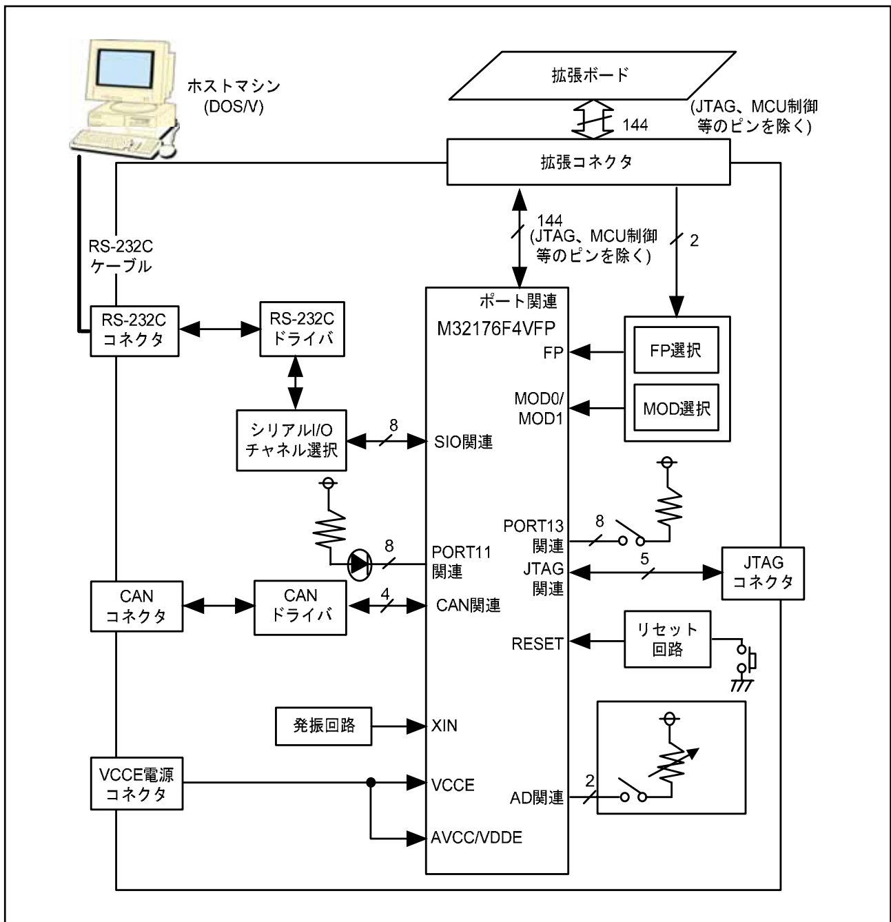
図 1.3 ブロック図
