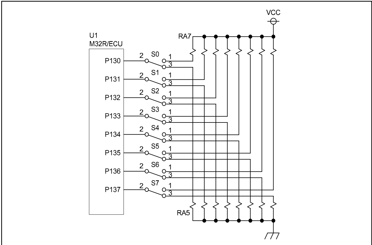
図 2.7 汎用入力ポート制御回路
