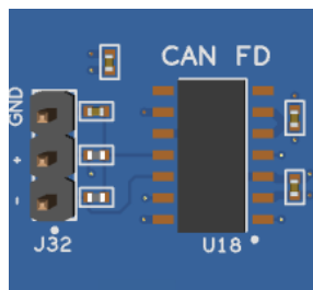
図 23. CAN バス
