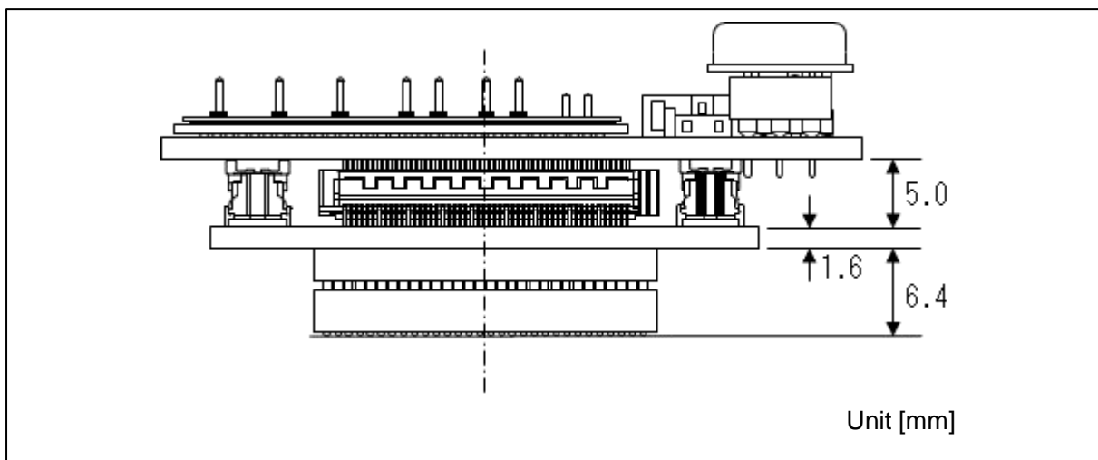
図 A-4. RTE7702012CBG468T000J 組立図 (468pin)
