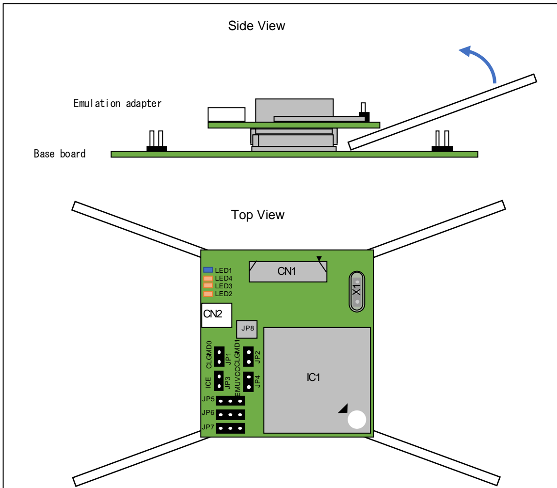
図 2-6 取り外し用スティック
