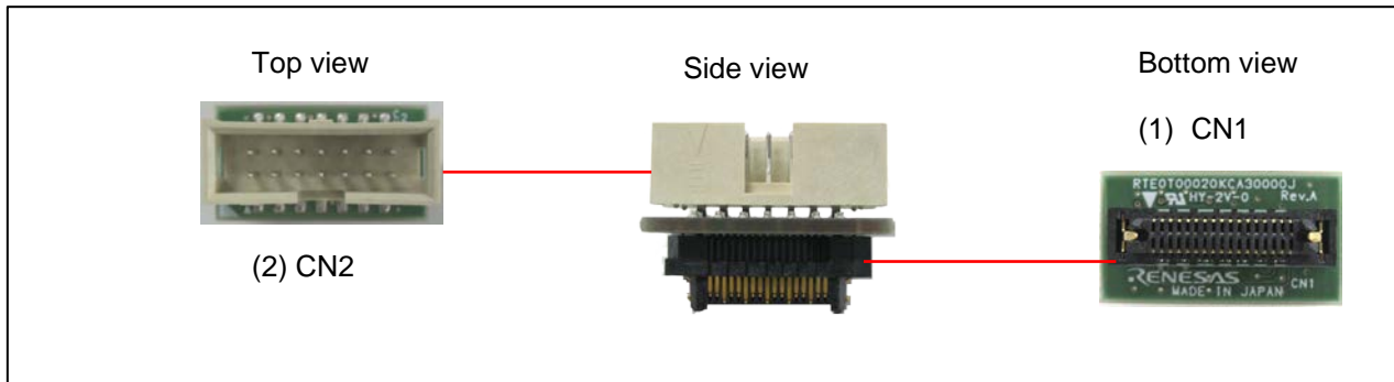
図 2-4 34 ピン-14 ピン変換アダプタ (RTE0T00020KCA30000J) 各部の名称
