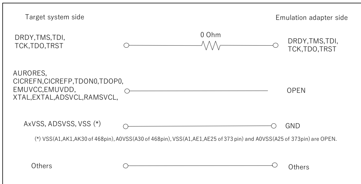
図 A-6. 等価回路
