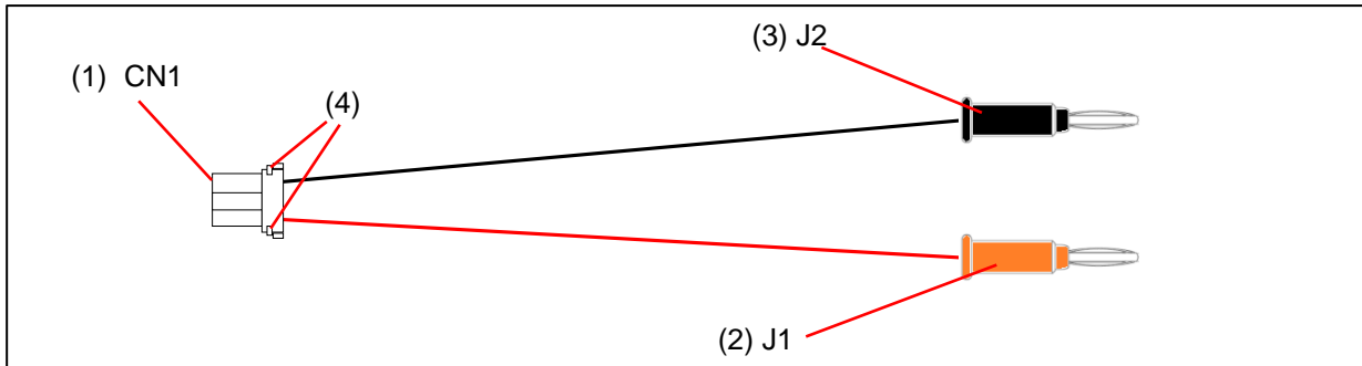
図 2-5 電源供給ケーブル各部の名称
