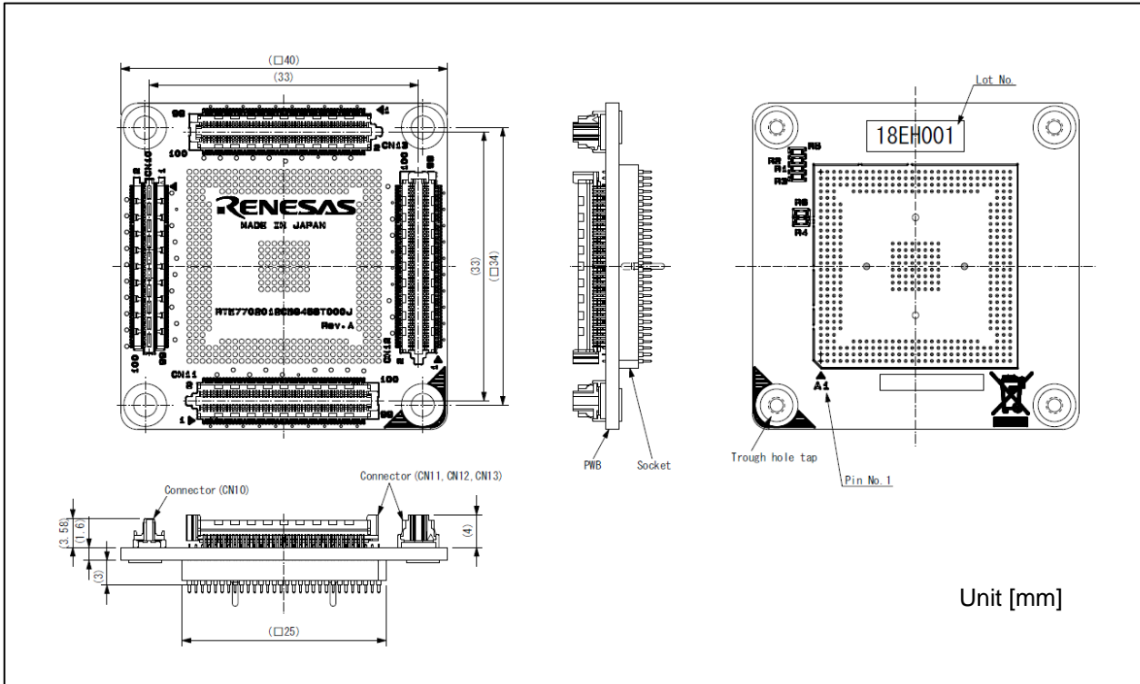
図 A-2. RTE7702012CBG468T000J 寸法図 (468pin)
