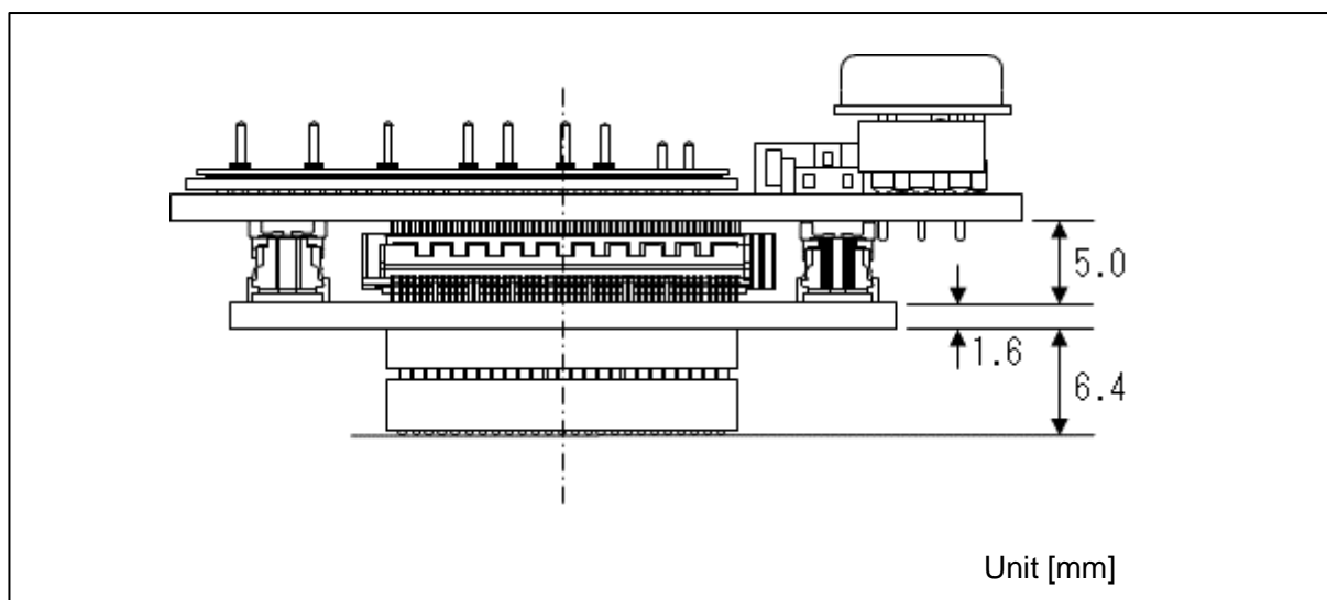
図 A-5. RTE7702011CBG373T000J 組立図 (373pin)
