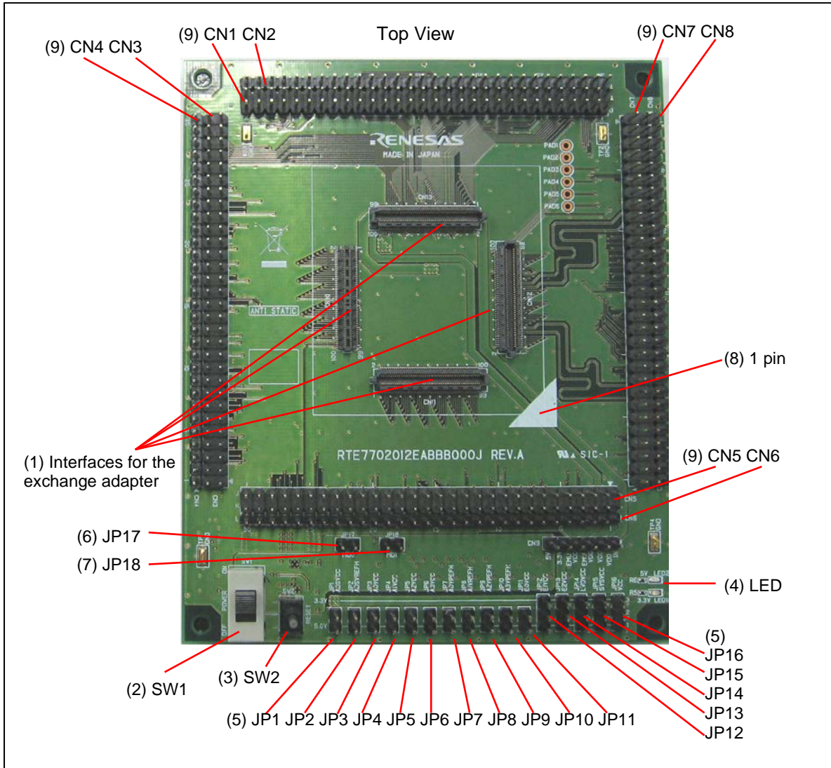
図 2-2 ベースボード (RTE7702012EABBB000J) 各部の名称
