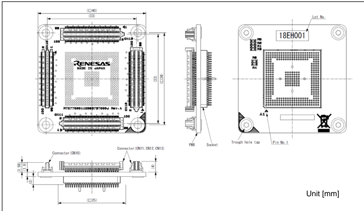
図 A-3. RTE7702011CBG373T000J 寸法図 (373pin)
