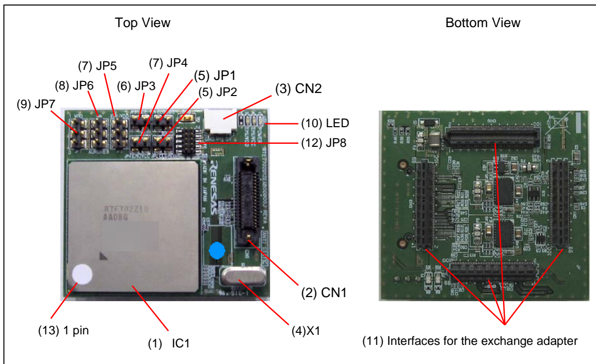
図 2-1 エミュレーションアダプタ (RTE7702012EAB00000J) 各部の名称
