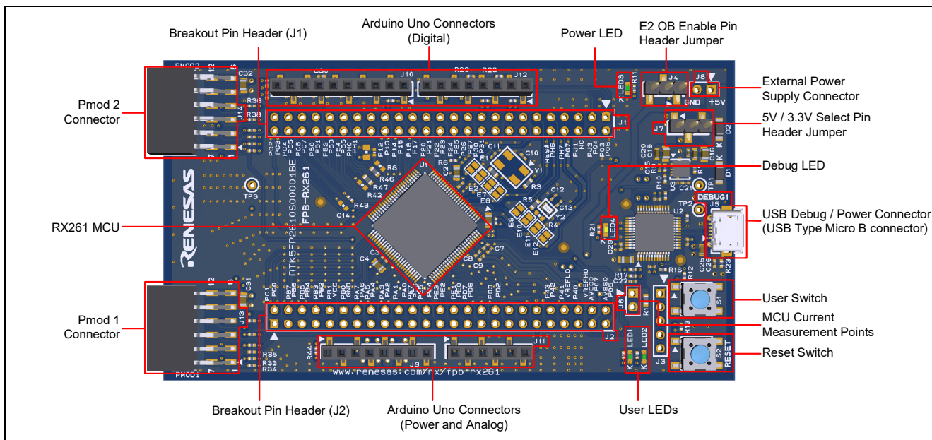
図 1 FPB-RX261 v1 (表面)
