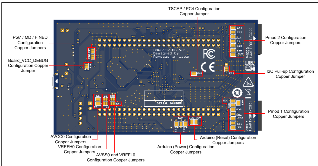
図 2 FPB-RX261 v1 (裏面)
