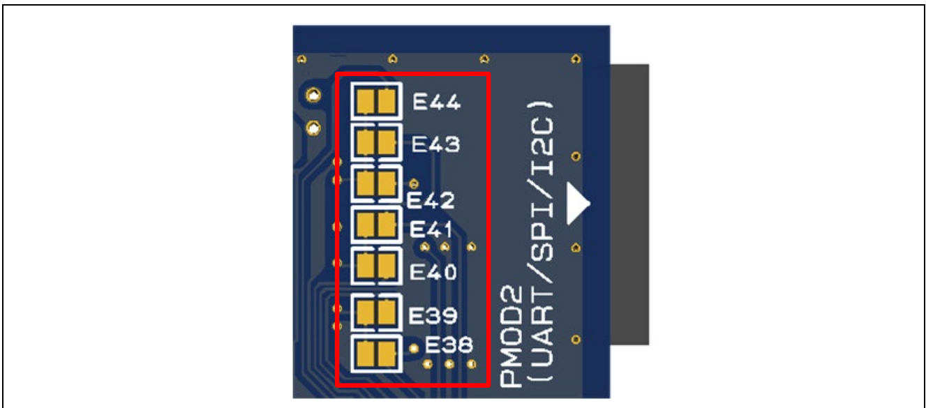
図 16 Pmod 2 はんだジャンパ (裏面)
