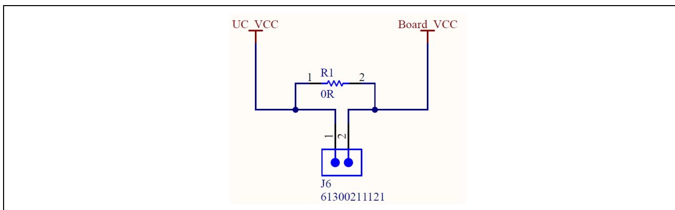
図 23 RX MCU 電流測定回路
