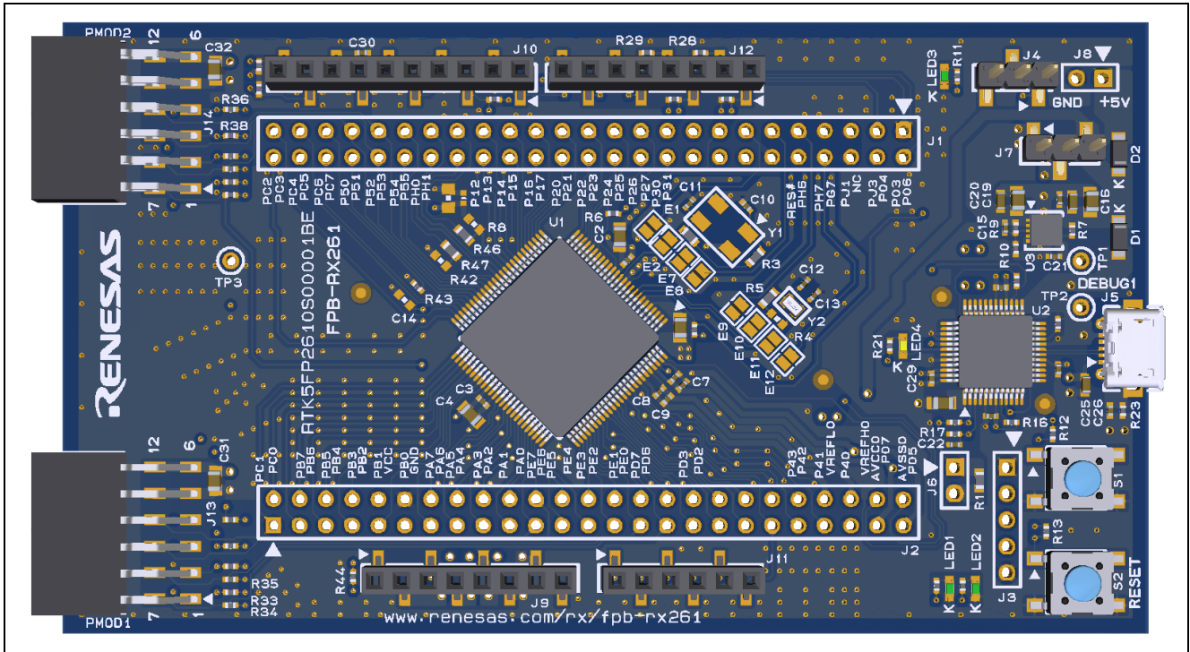
図 3 FPB-RX261 v1
