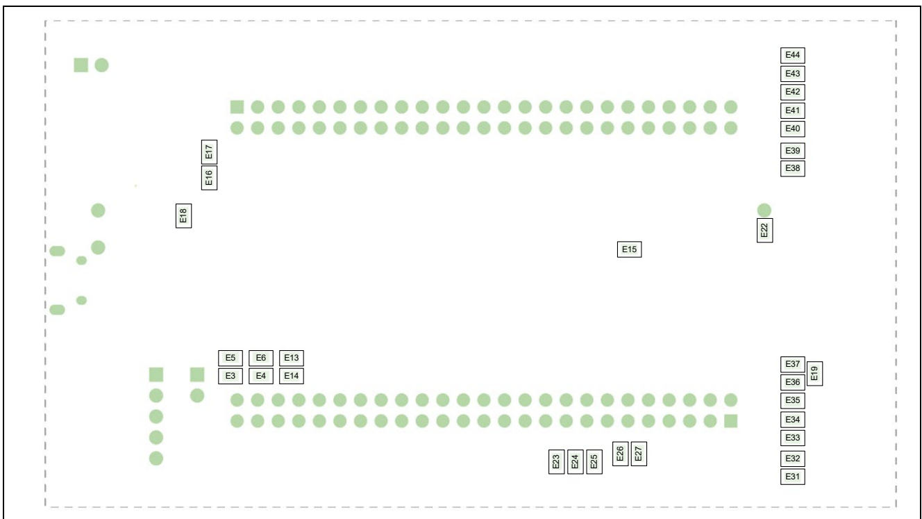
図 6 部品のリファレンス番号 (裏面)
