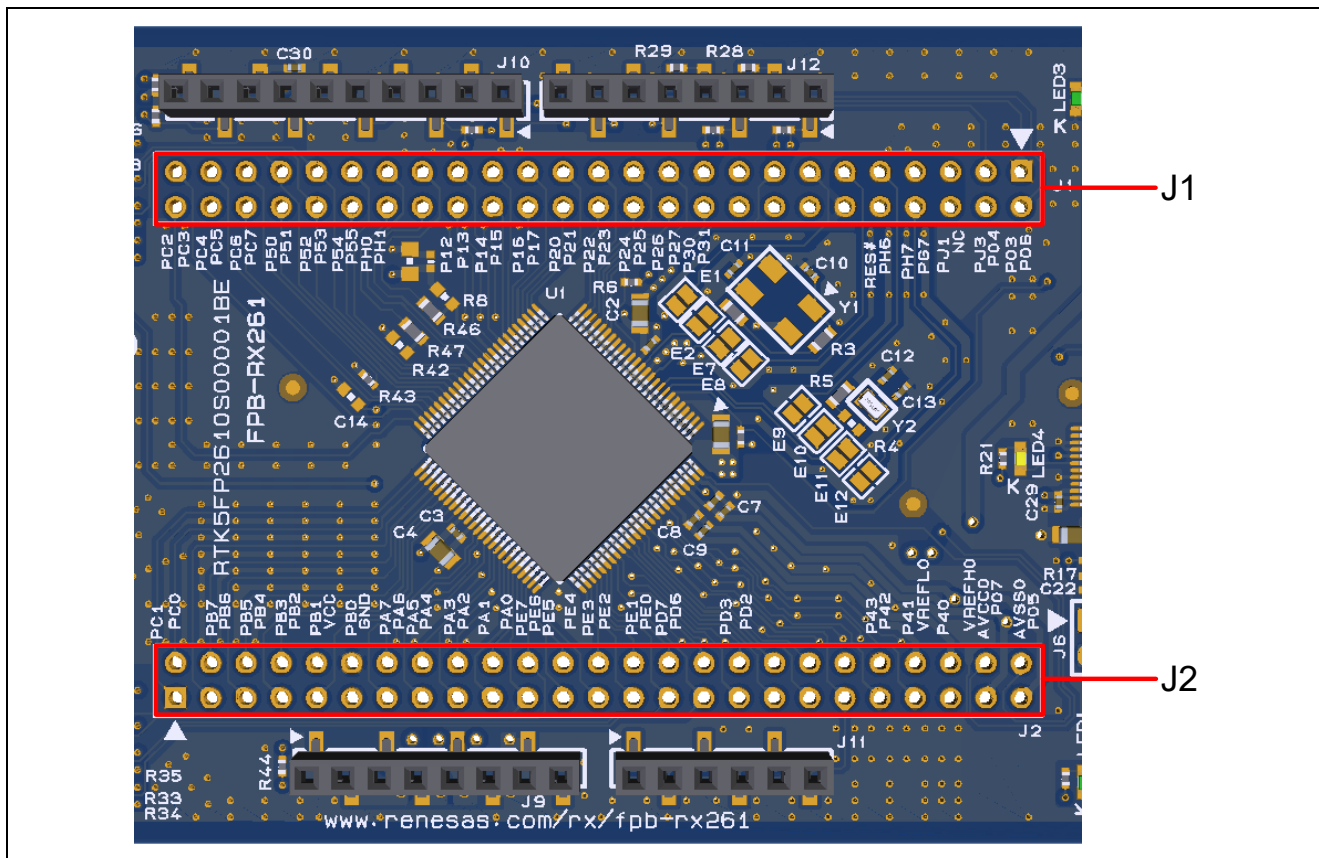
図 22 ブレイクアウトピンヘッダ J1 および J2
