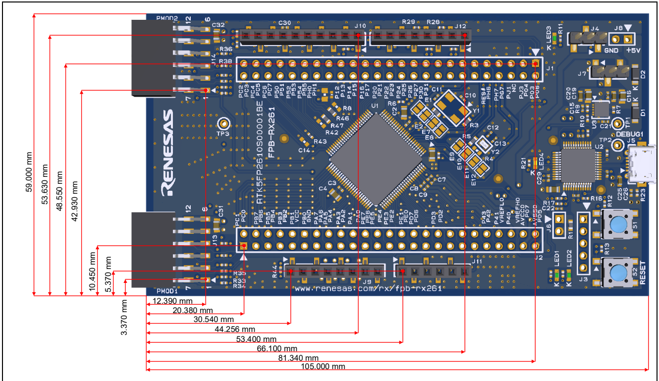
図 7 寸法図
