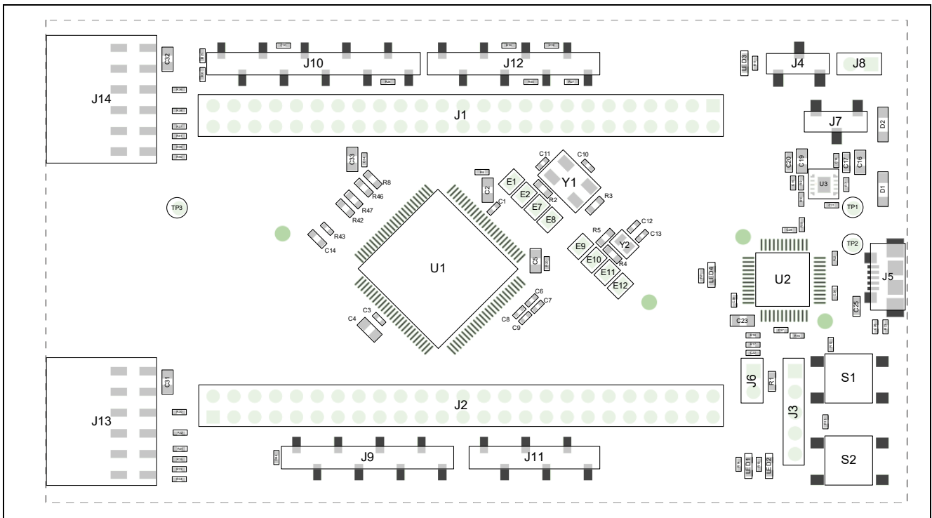
図 5 部品のリファレンス番号 (表面)
