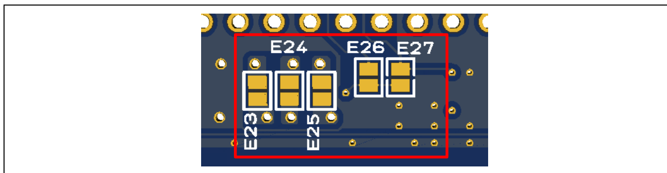
図 18 Arduino Uno はんだジャンパ (裏面)
