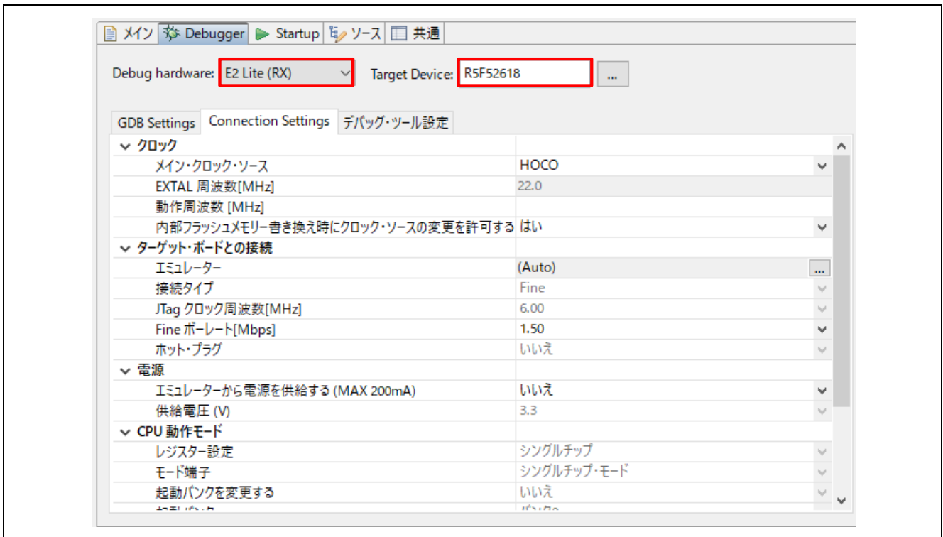
図 11 e 2 Studio の設定
