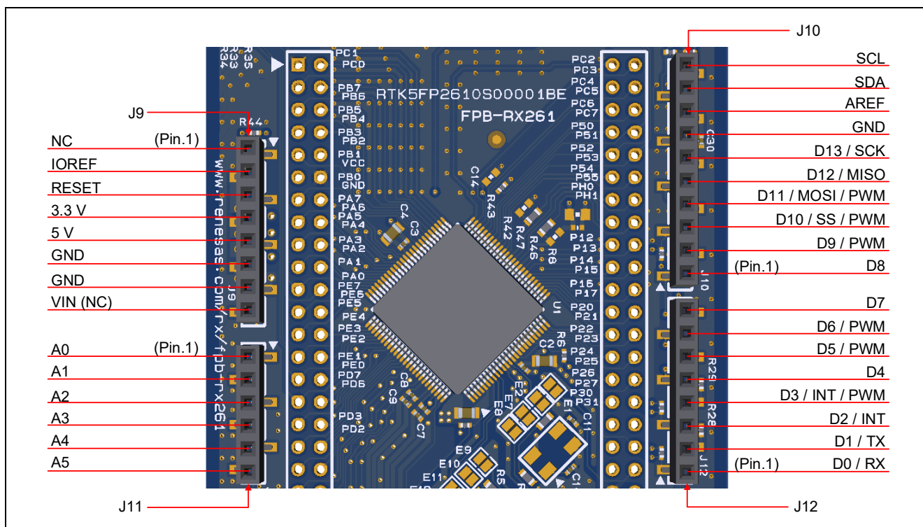
図 17 Arduino Uno コネクタ
