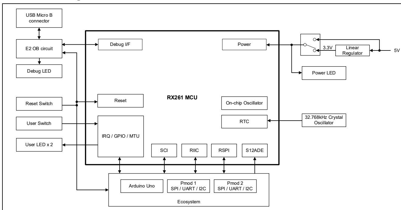
図 4 FPB-RX261 v1 のブロック図
