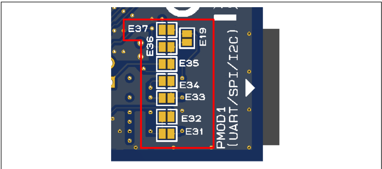
図 14 Pmod 1 はんだジャンパ (裏面)
