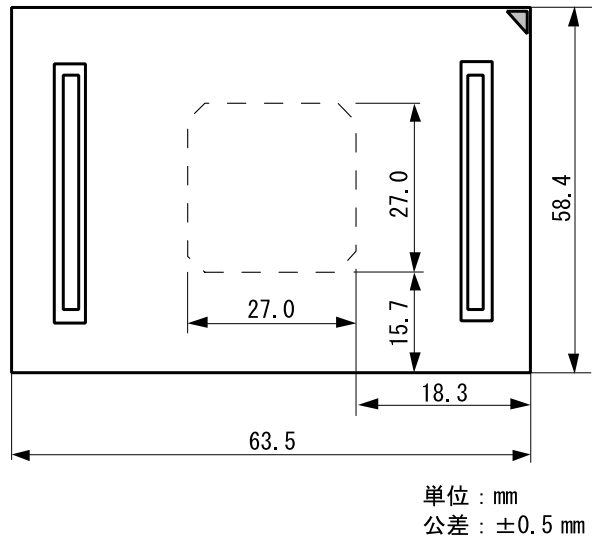
図 6 ケーブル先端部の寸法
