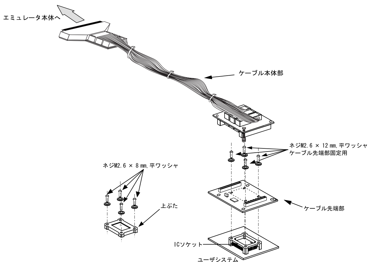
図 1 HS38024ECN61H ユーザシステムインタフェースケーブル
