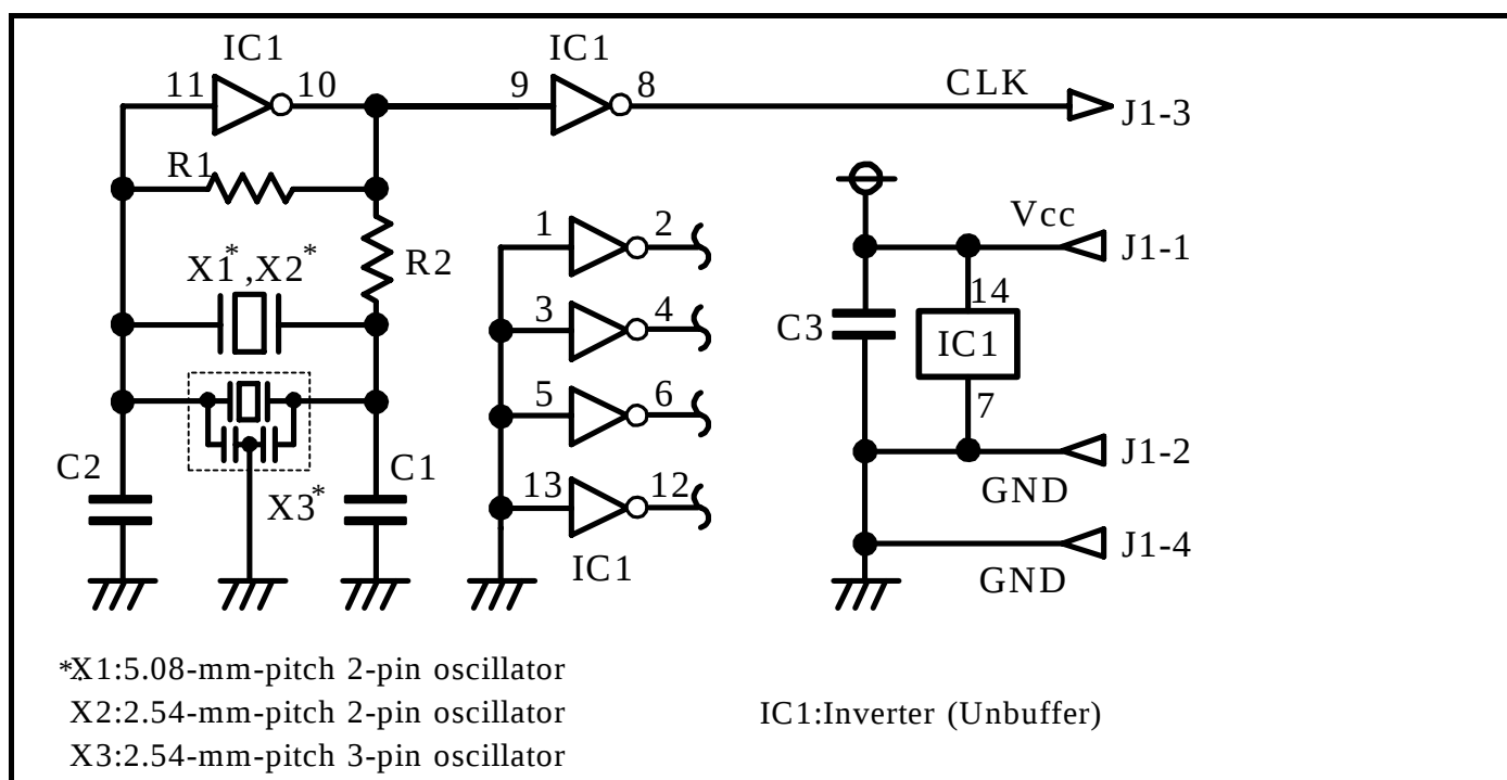
図 2.14 発振回路基板ベアボードOSC-2の回路図
