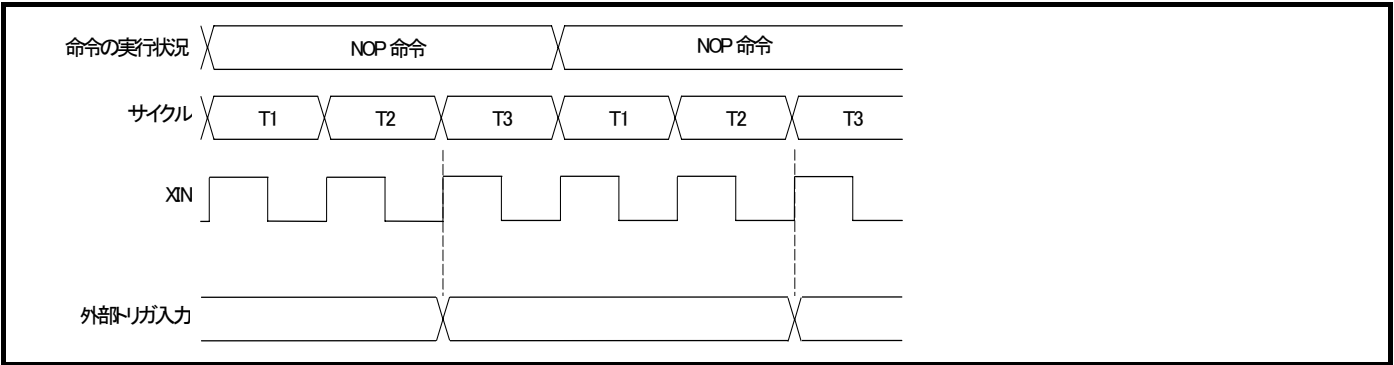
図 2.18 外部トリガ入力タイミング
