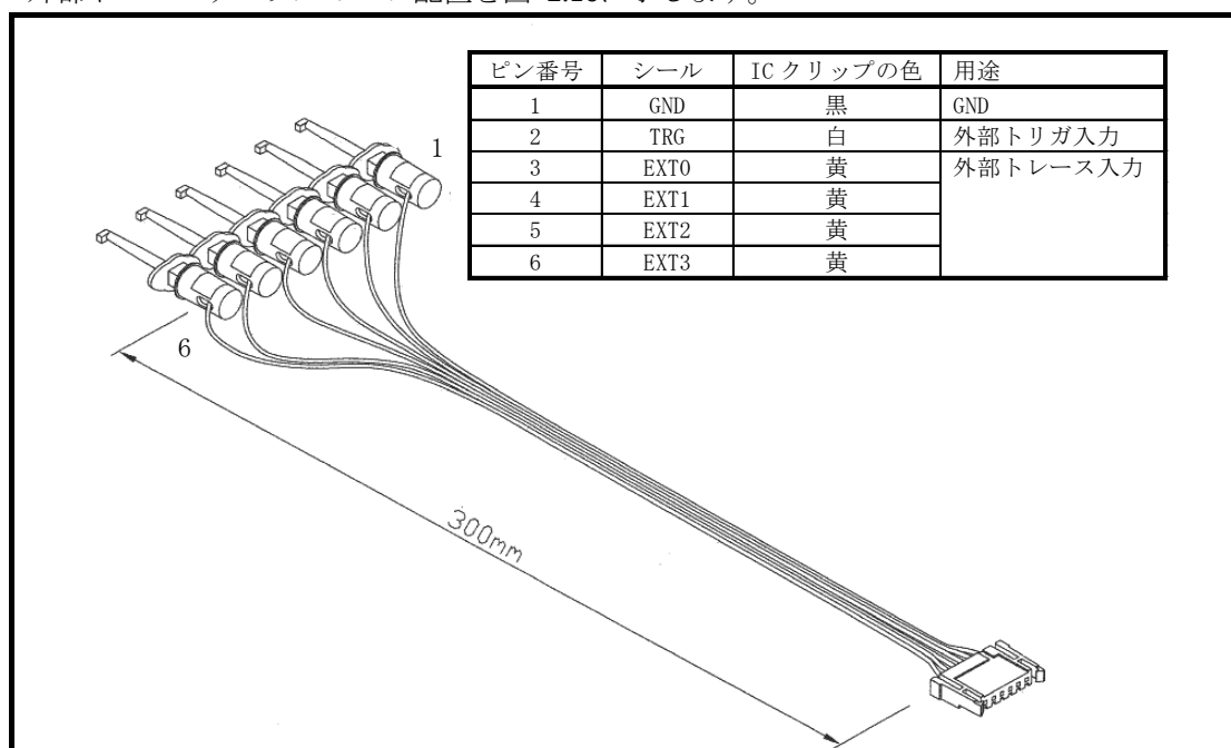
図 2.16 外部トレースケーブルのピン配置
