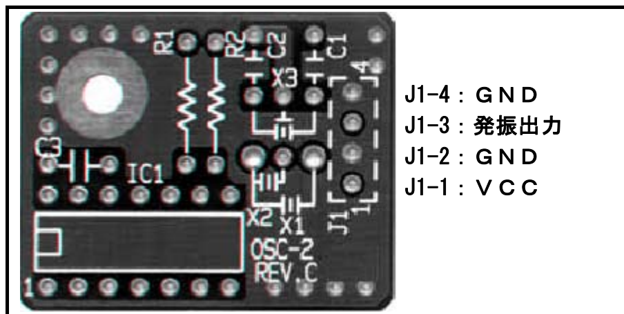
図 2.13 発振回路基板ベアボードOSC-2の外形とコネクタピン配置
