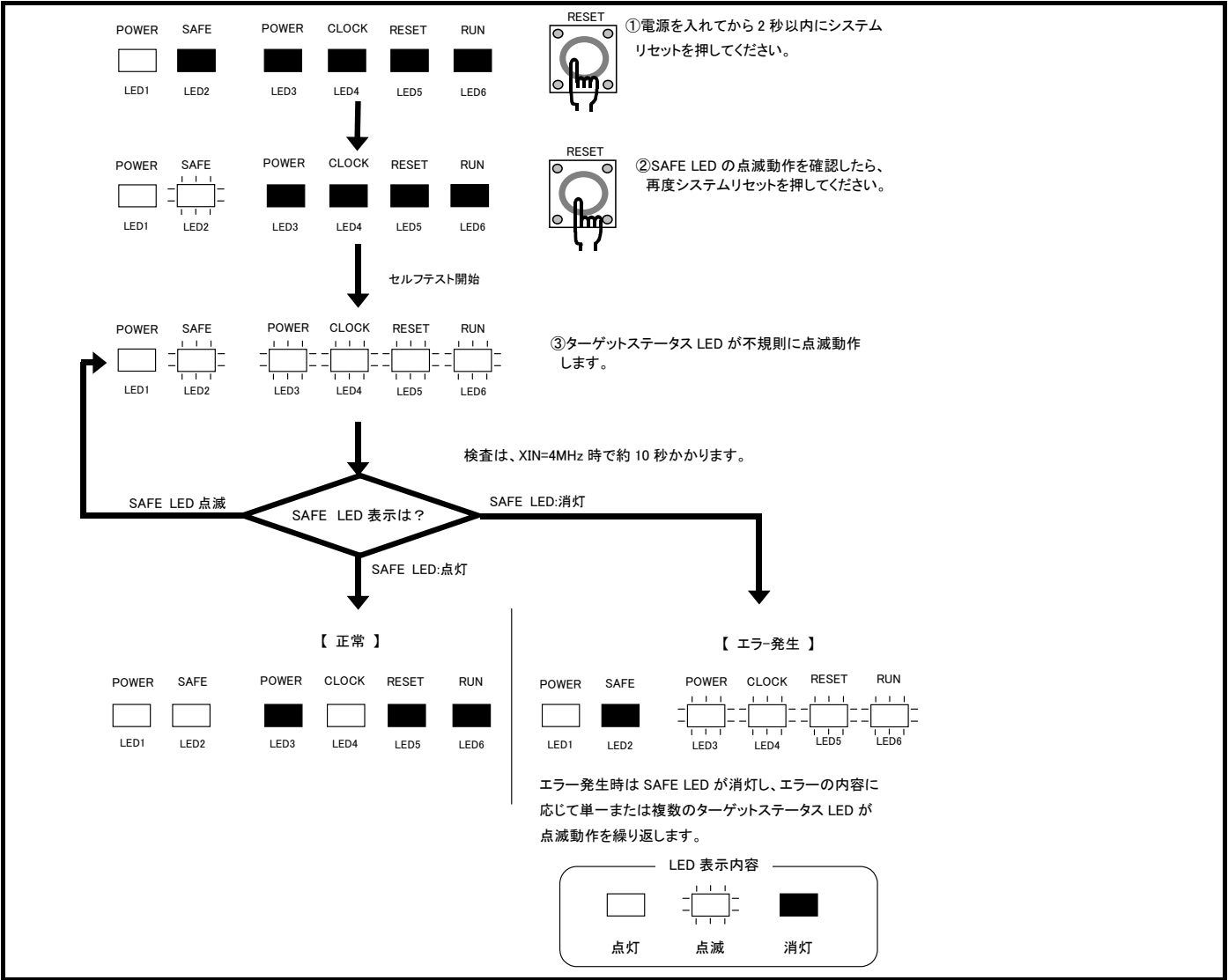
図 2.9 セルフチェック時のLED表示
