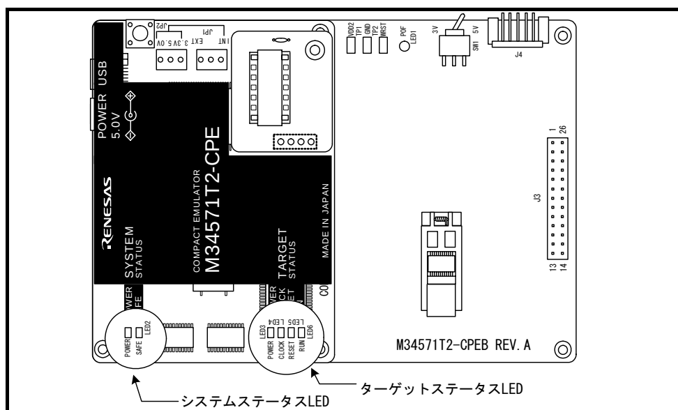
図 2.6 システムステータスLEDとターゲットステータスLEDの位置
