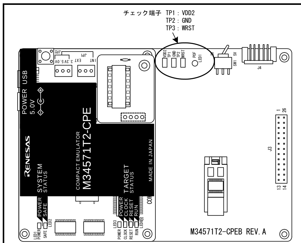
図 2.19 チェック端子の位置
