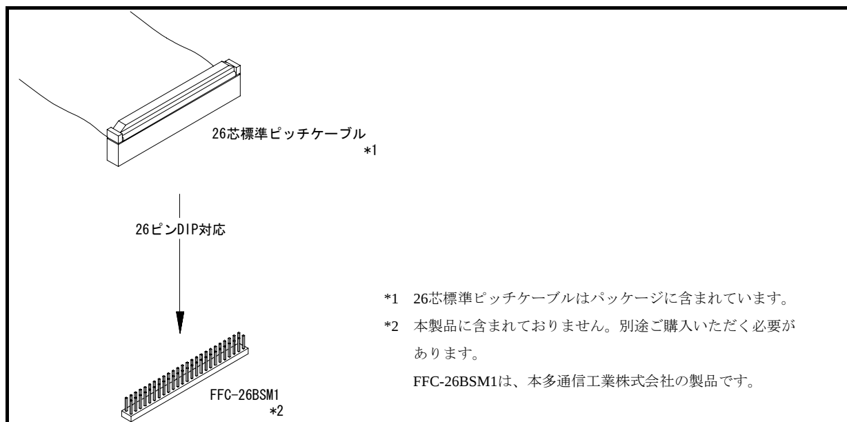
図 2.10 ユーザシステムとの接続
