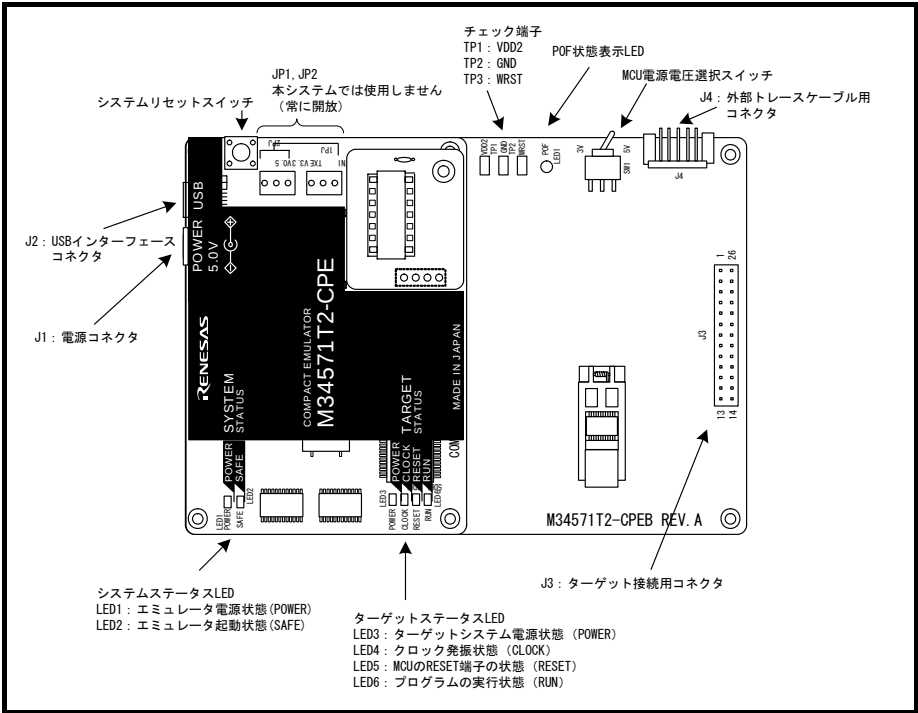
図 1.2 エミュレータ各部の名称(M34571T2-CPE上面)
