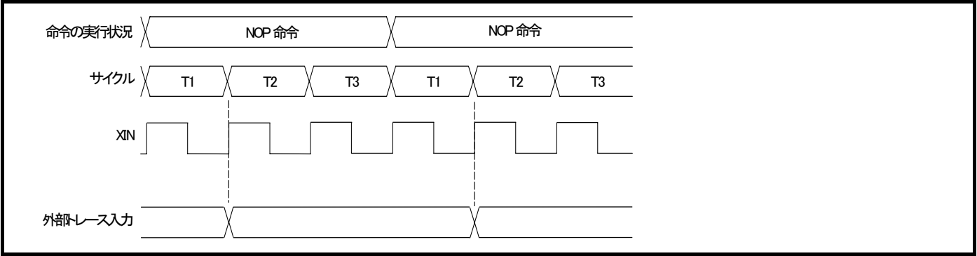
図 2.17 外部トレース入力タイミング
