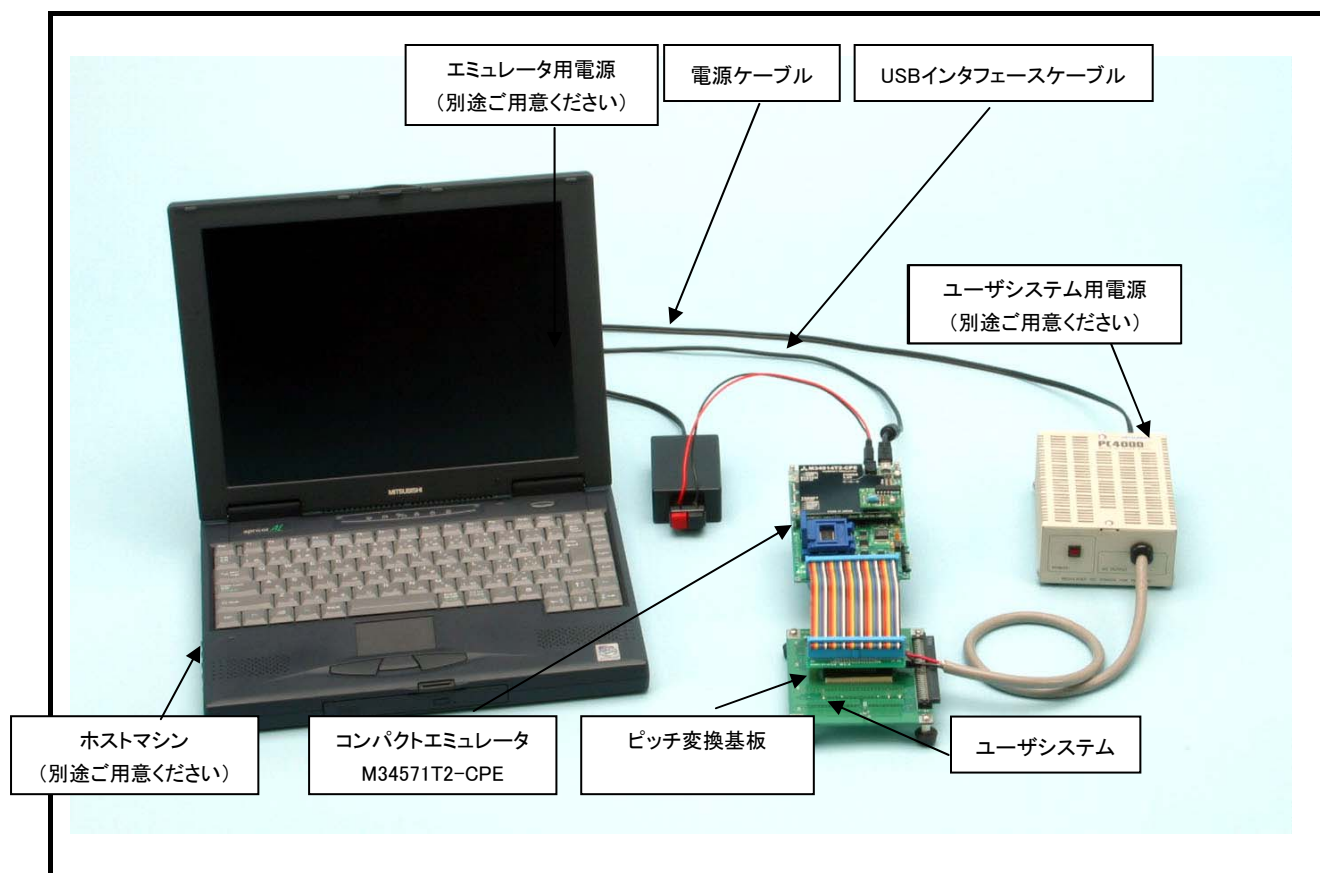
図 1.1 システム構成図
