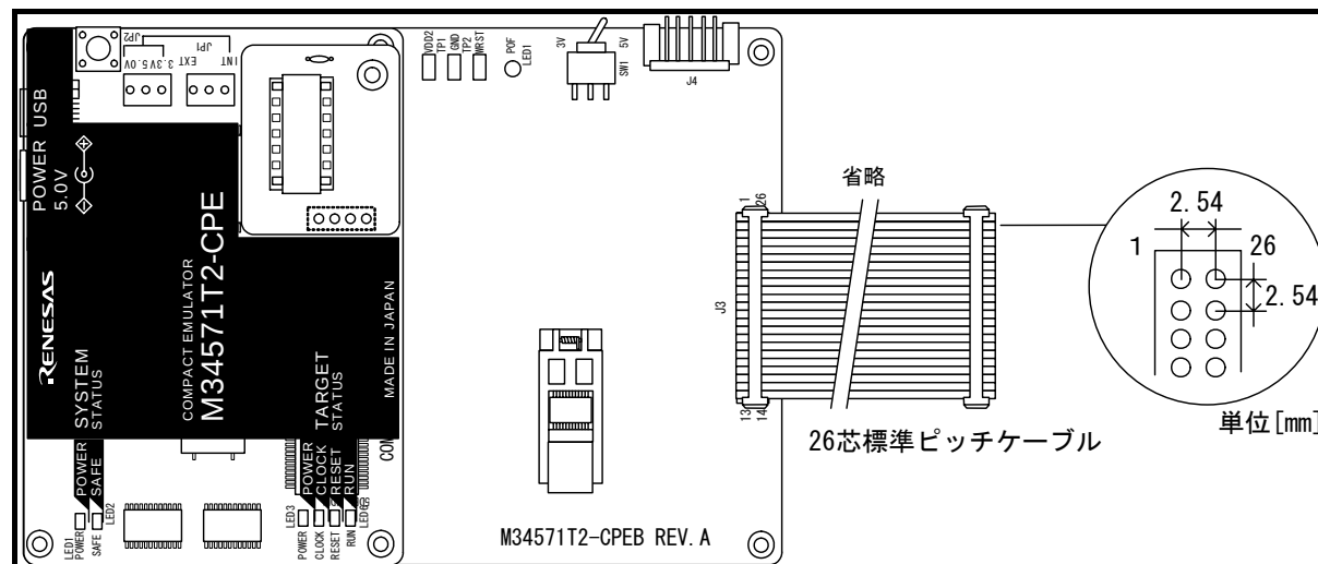
図 2.11 26ピン2.54mmピッチユーザシステムへの接続
