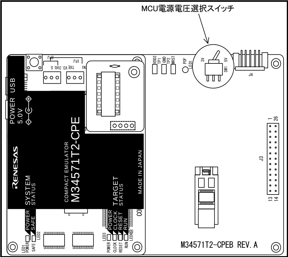
図 2.5 エミュレータのスイッチ位置
