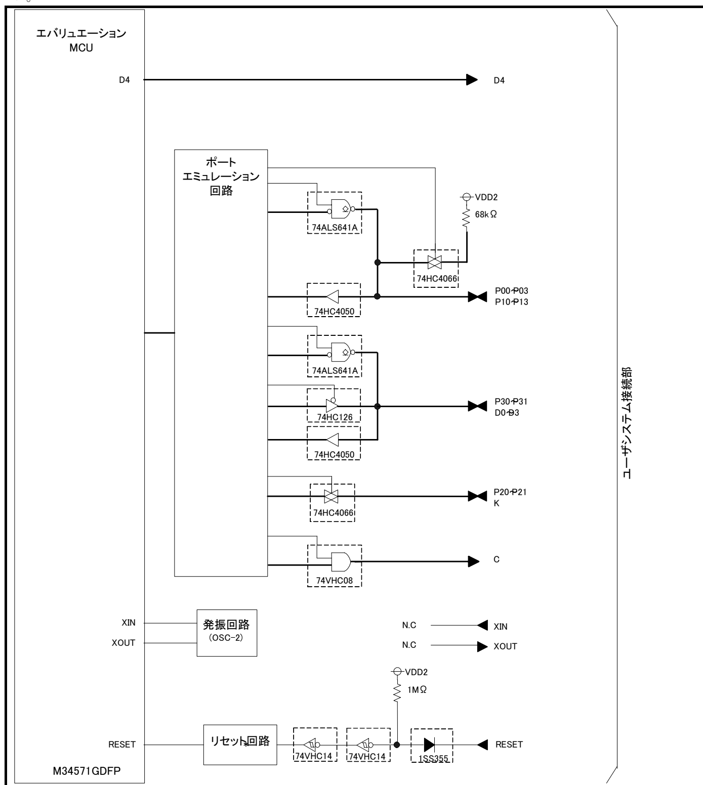
図 4.2 M34571T2-CPEの接続図(一部)
