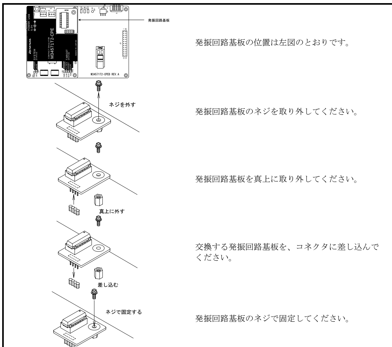
図 2.12 発振回路基板の交換手順
