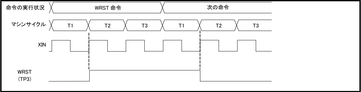
図 2.20 チェック端子WRSTの出力波形
