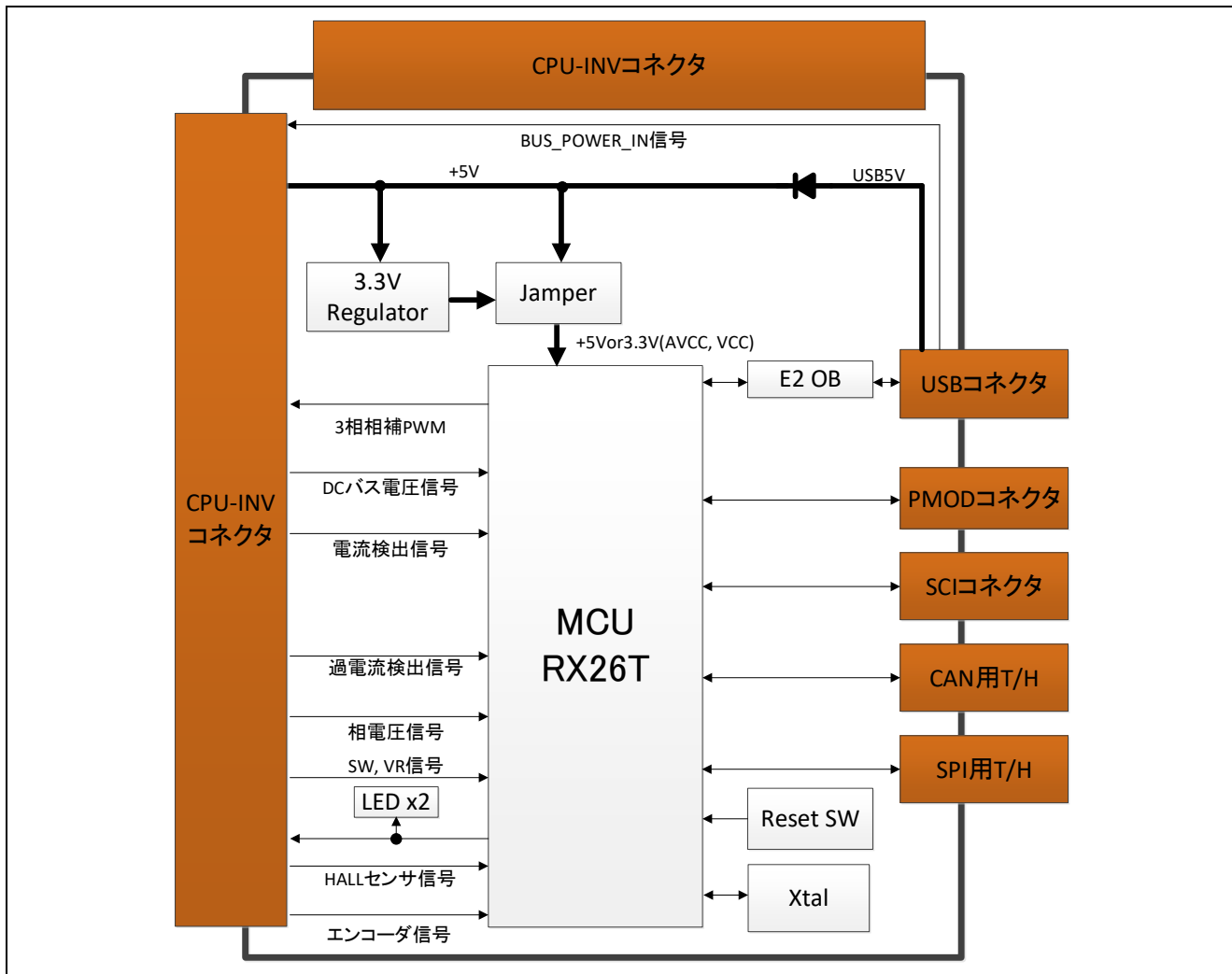
図 4-1 CPU ボードのブロック図
