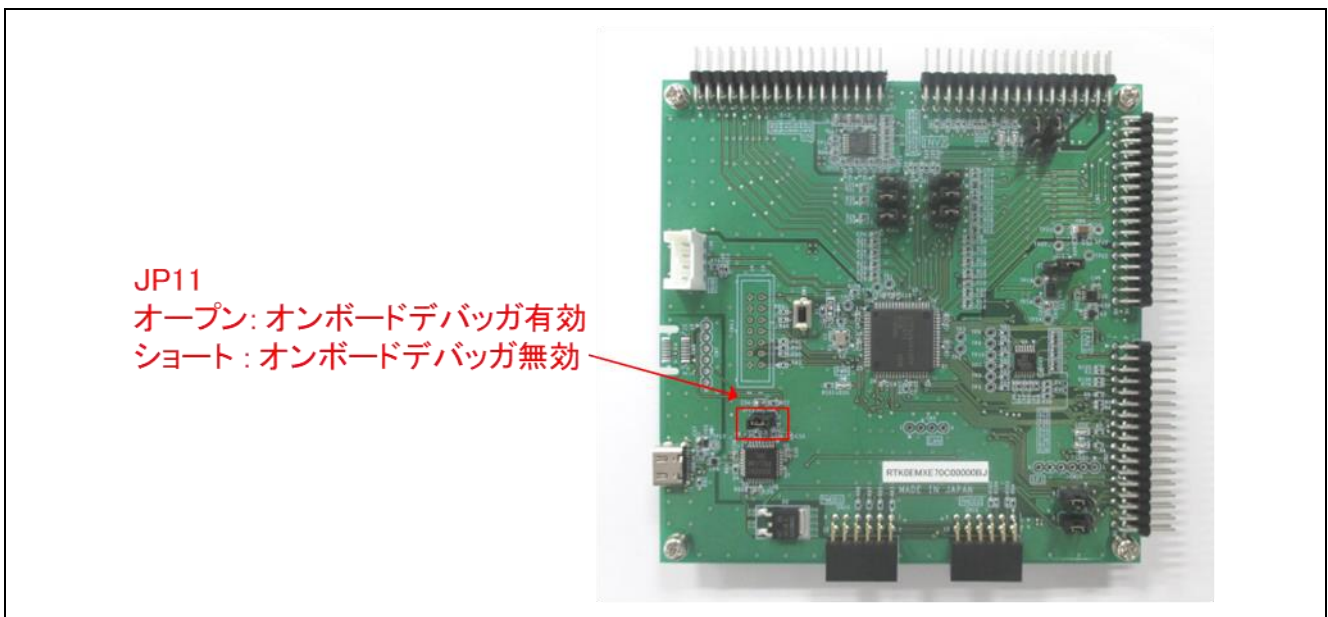
図 5-1 ジャンパJP11の設定
