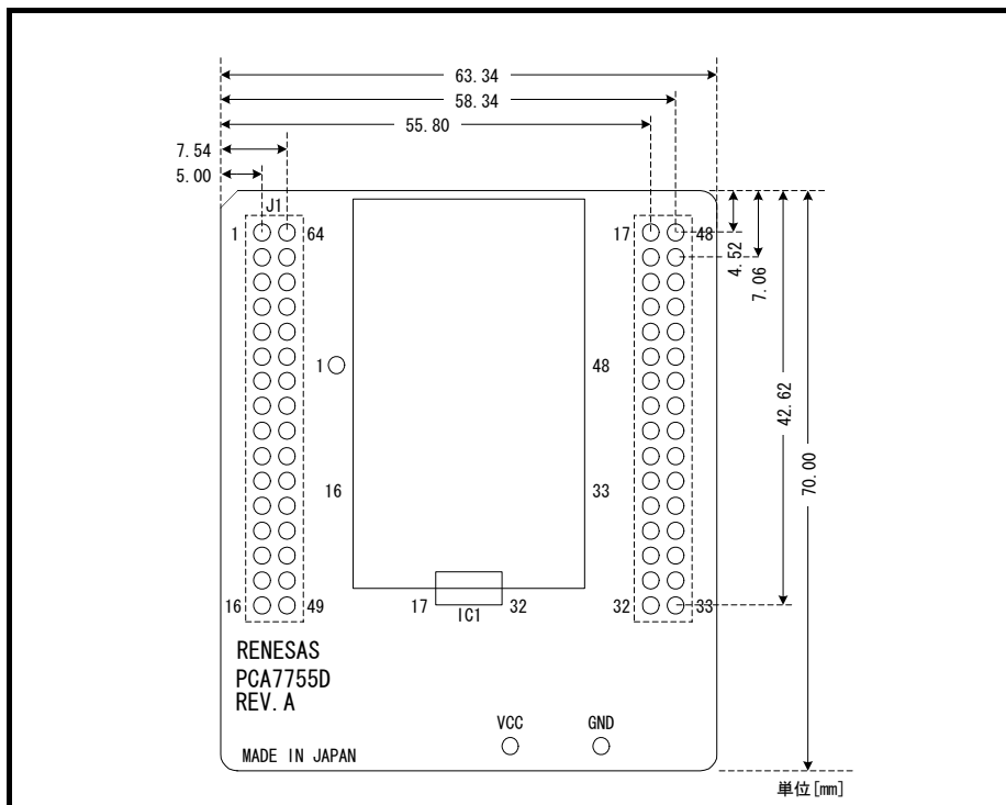
図6 PCA7755D寸法図
