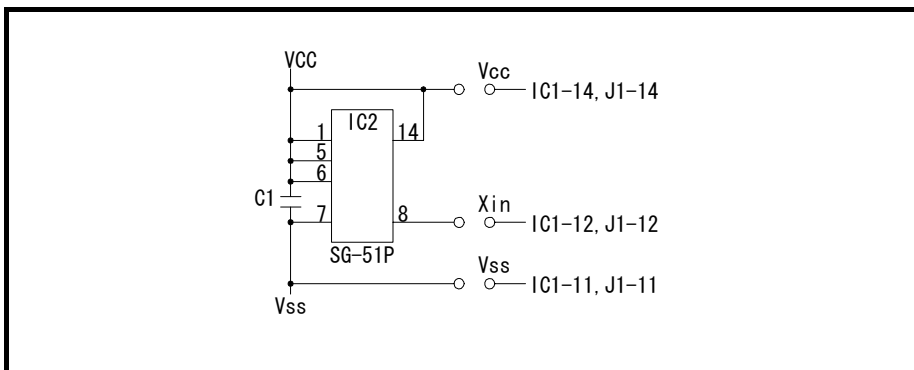
図3 IC1使用時の接続図
