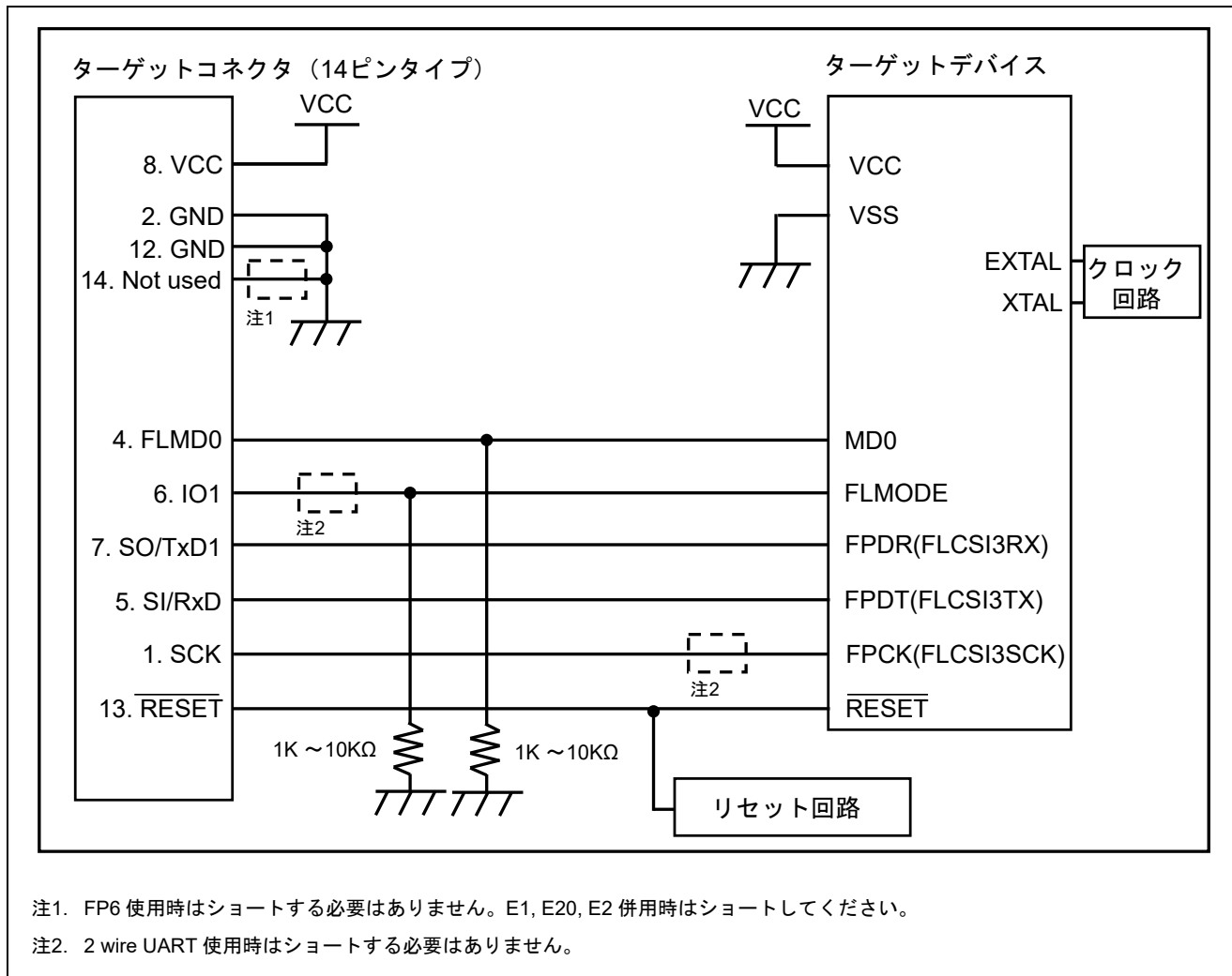
図 3.10 2 wire UART または CSI (RH850ファミリ) の回路例 (RH850/E1xの回路例)
