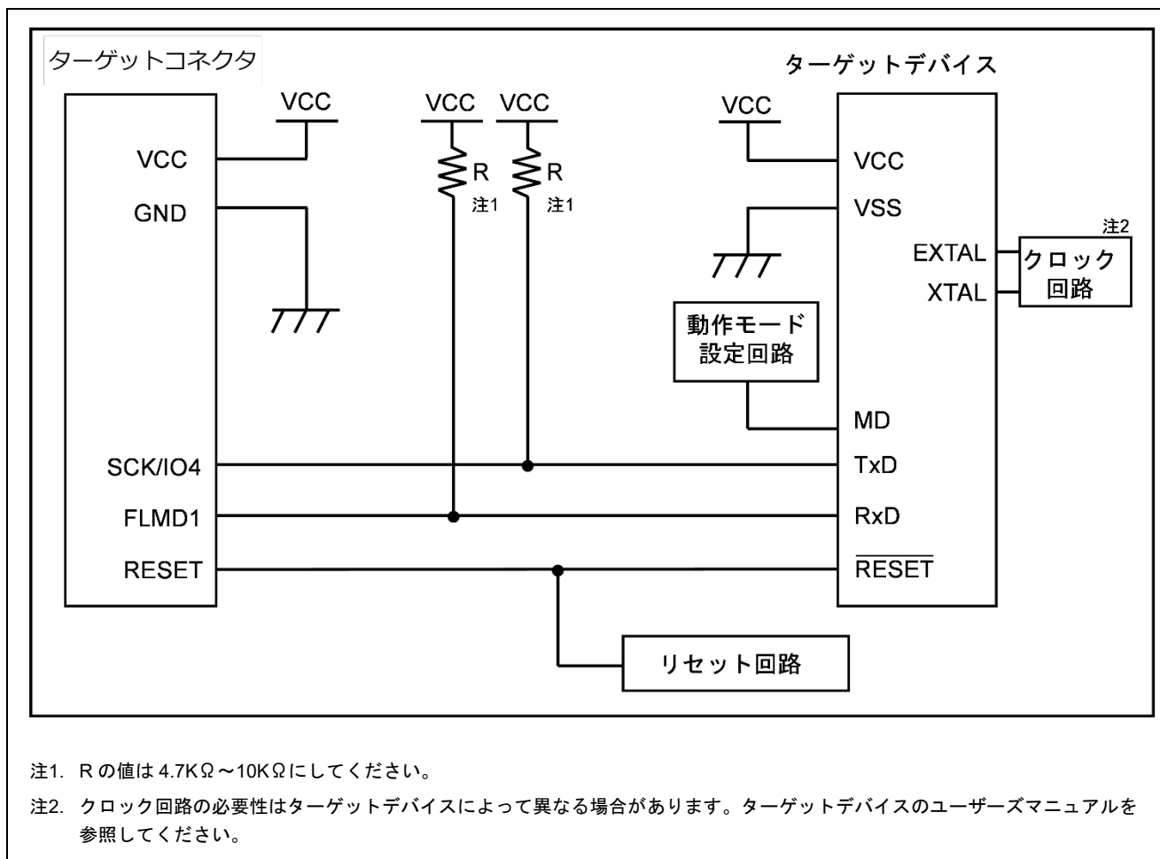
図 3.12 UARTの回路例 (R7F0E017Dの回路例)
