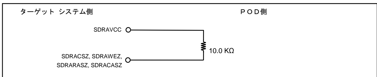
図 A-15 等価回路O
