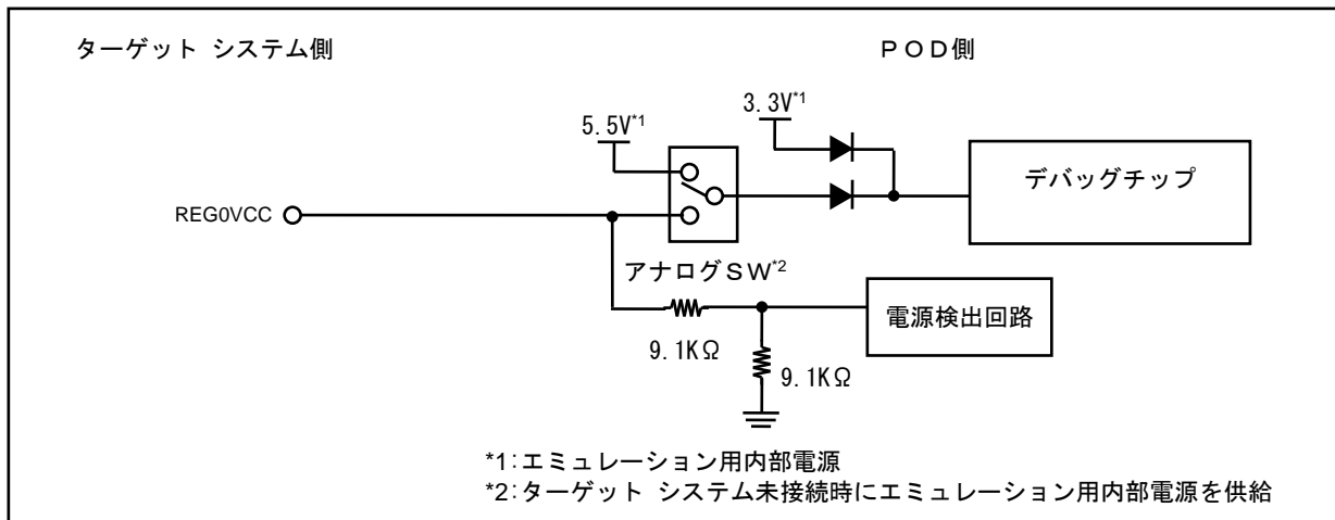
図 A-5 等価回路E
