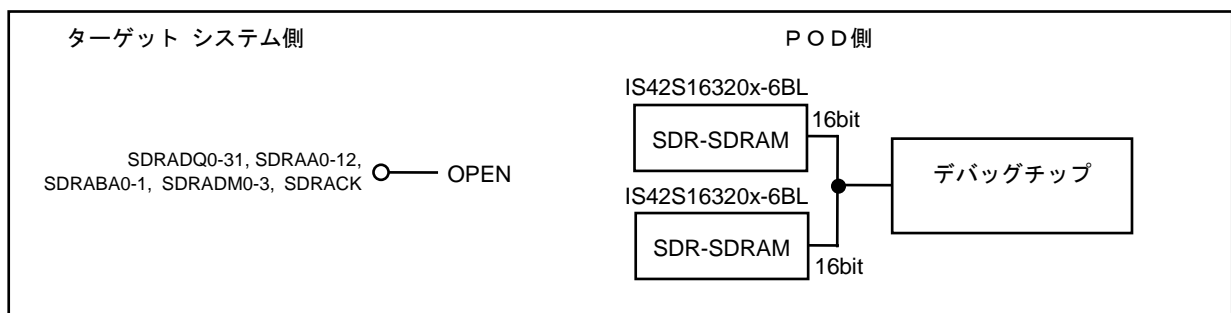
図 A-16 等価回路P
