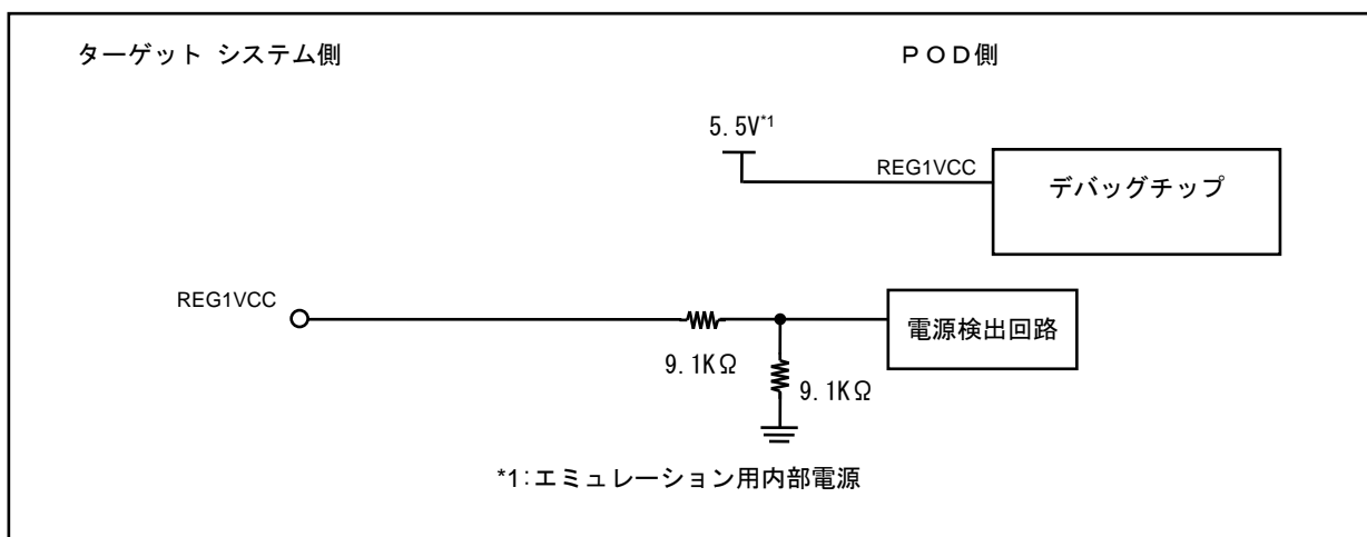
図 A-6 等価回路F
