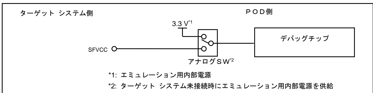
図 A-2 等価回路B
