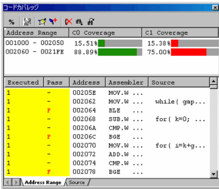
図 5.76 [コードカバレッジ] ウィンドウ (アドレス指定)
