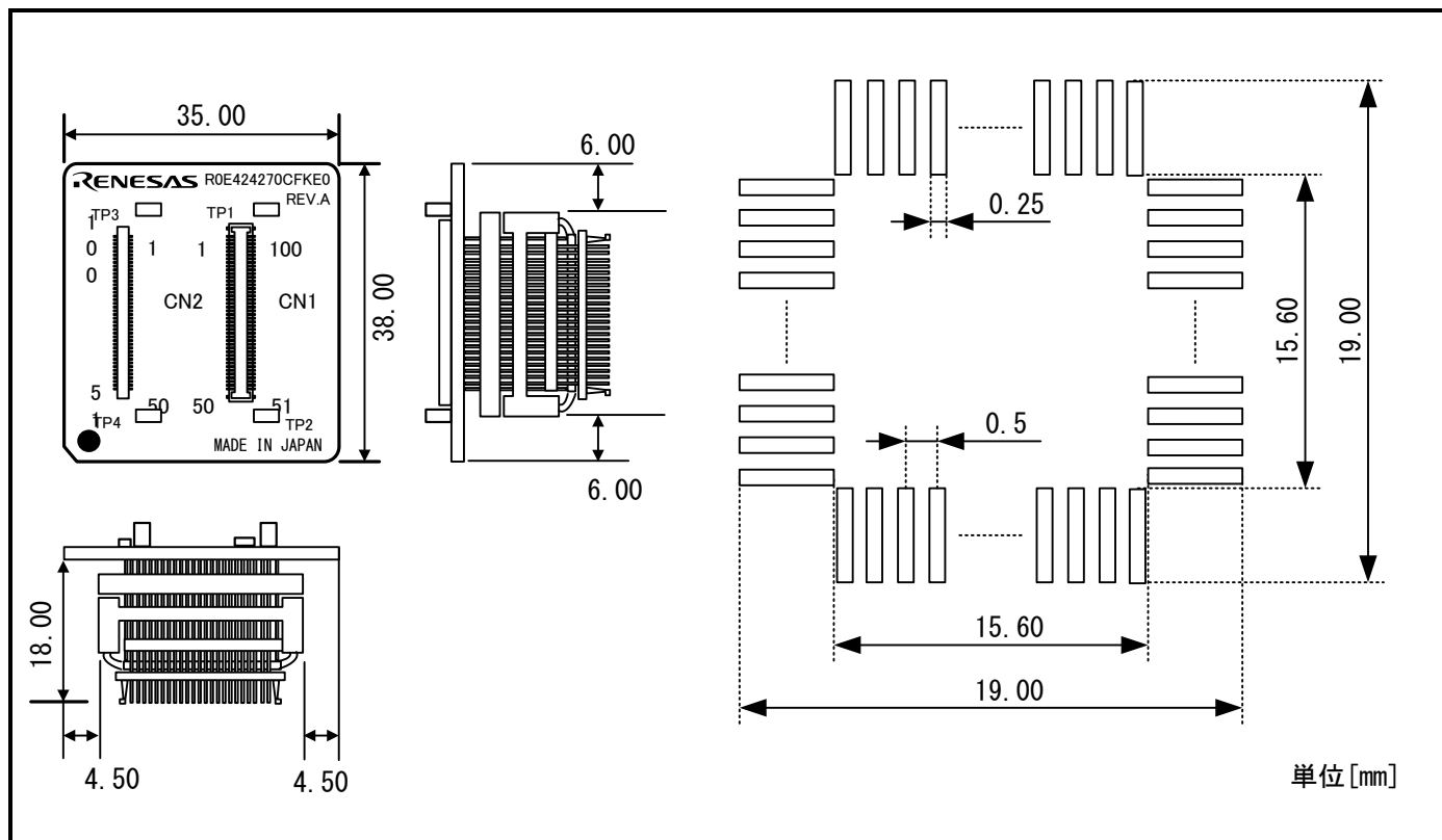
図7.4 R0E424270CFKE0ユーザーシステム接続部の寸法図および参考フットパターン
