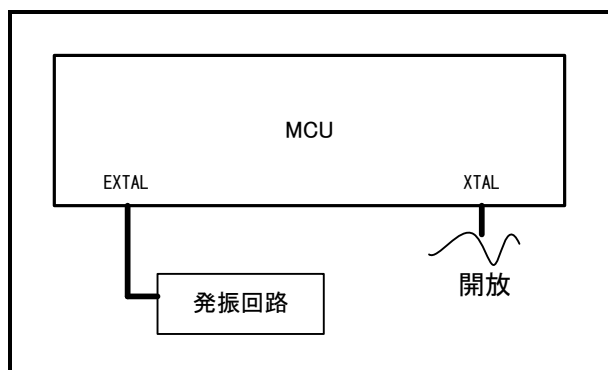
図2.8 ユーザシステム上発振回路の使用
