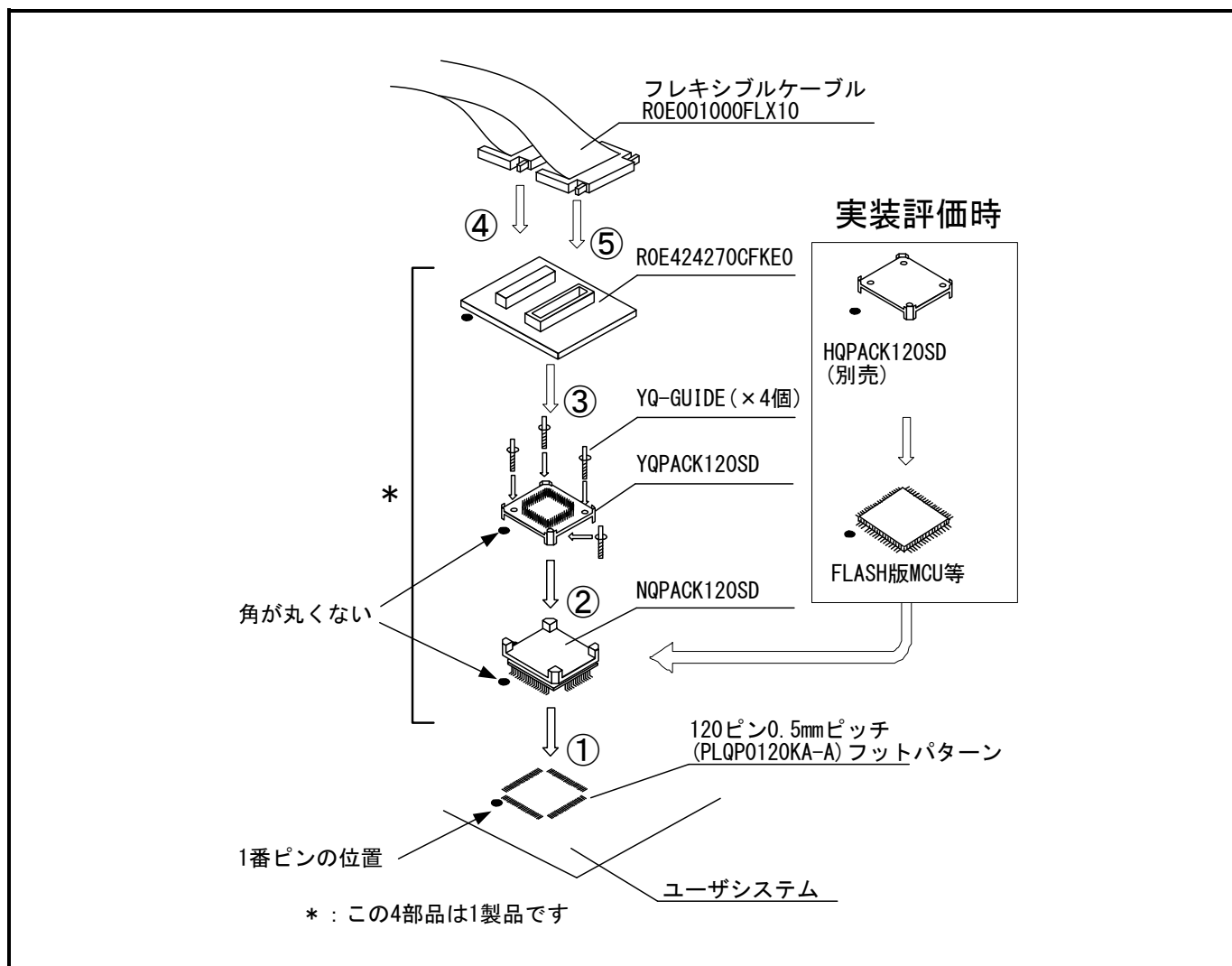
図2.12 120ピン0.5mmピッチフットパターンへの接続
