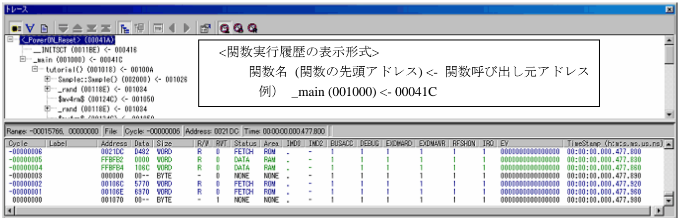
図3.38 [トレース]ウィンドウ (関数実行履歴—解析後)
