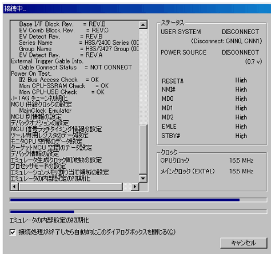
図5.6 [接続] ダイアログボックス
