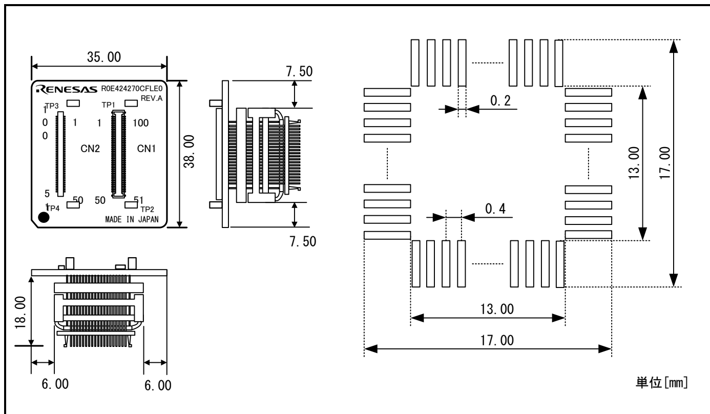
図7.3 R0E424270CFLE0ユーザーシステム接続部の寸法図および参考フットパターン
