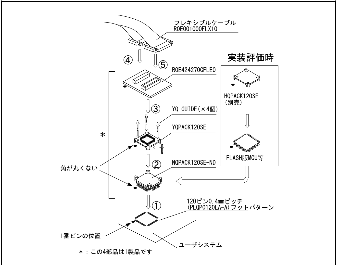
図2.11 120ピン0.4mmピッチフットパターンへの接続
