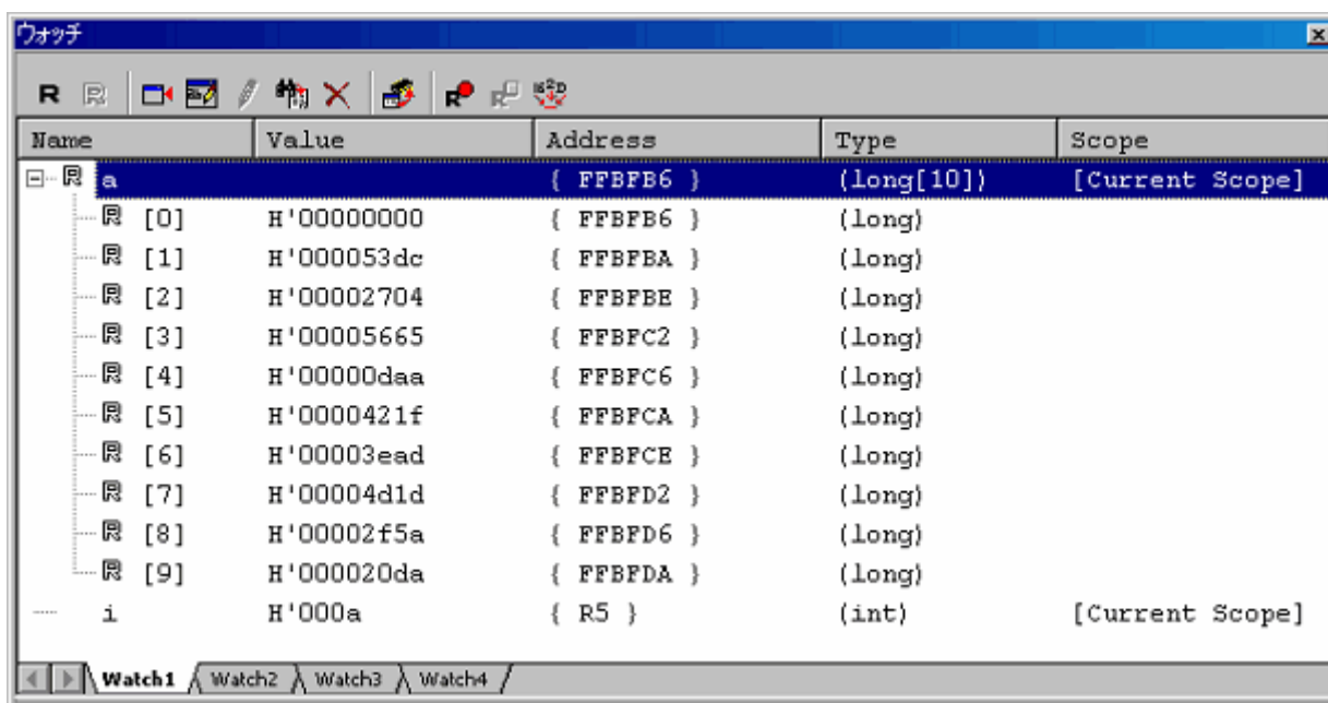
図3.17 [ウォッチ]ウィンドウ (配列要素の表示)
