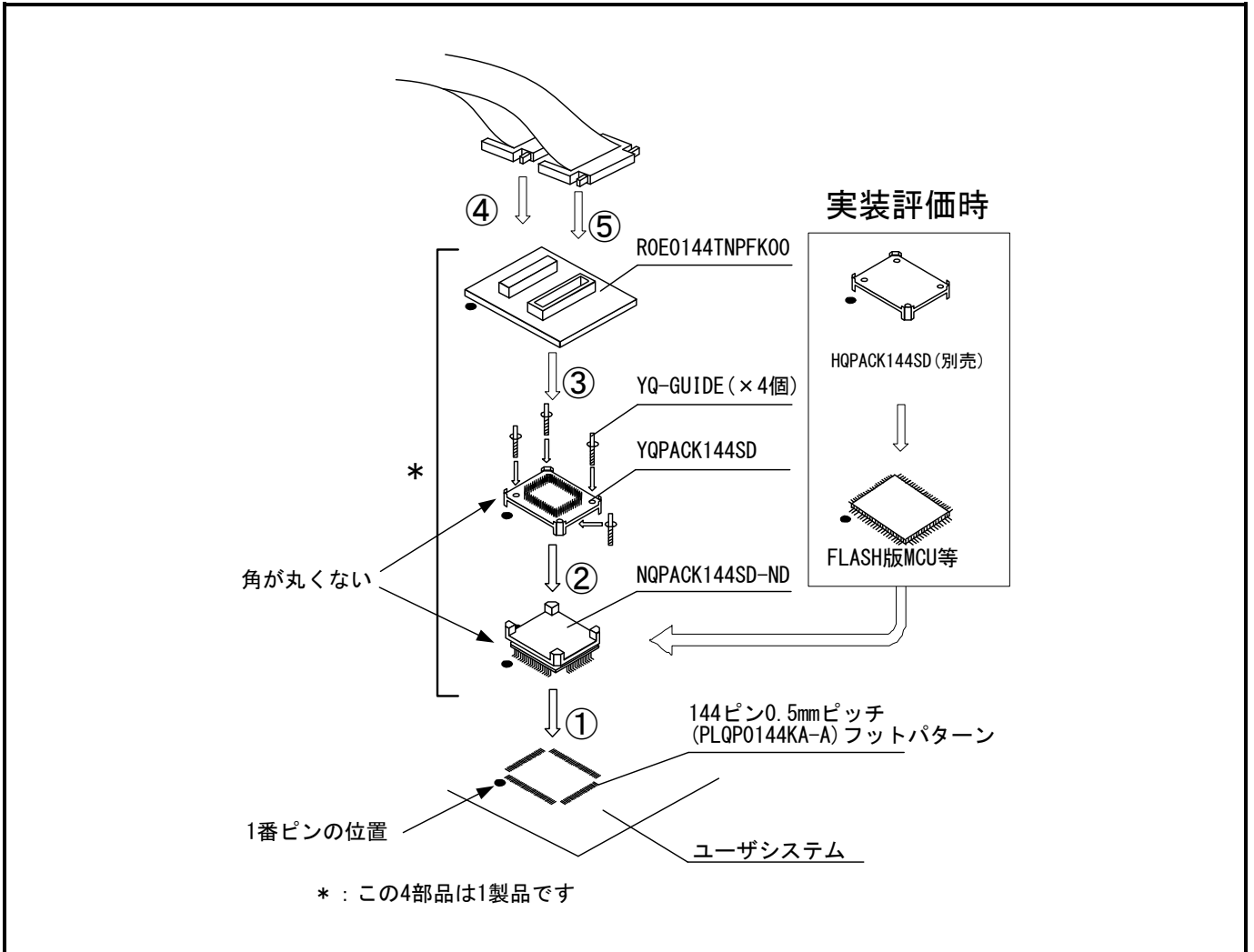
図2.13 144ピン0.5mmピッチフットパターンへの接続
