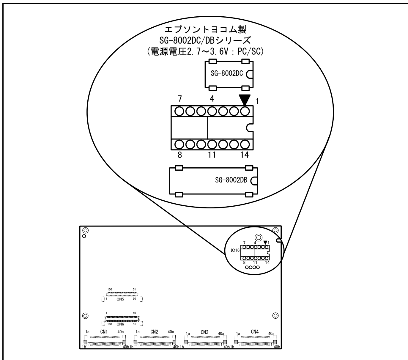
図2.7 発振モジュール交換
