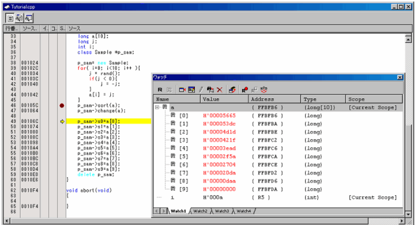
図3.24 [エディタ]ウィンドウ (ステップオーバー)
