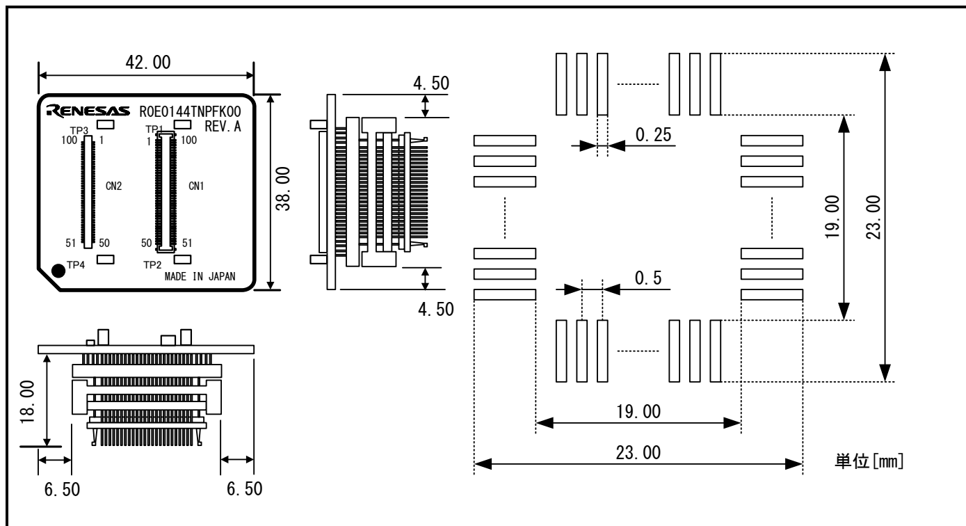
図7.5 R0E0144TNPFK00ユーザーシステム接続部の寸法図および参考フットパターン
