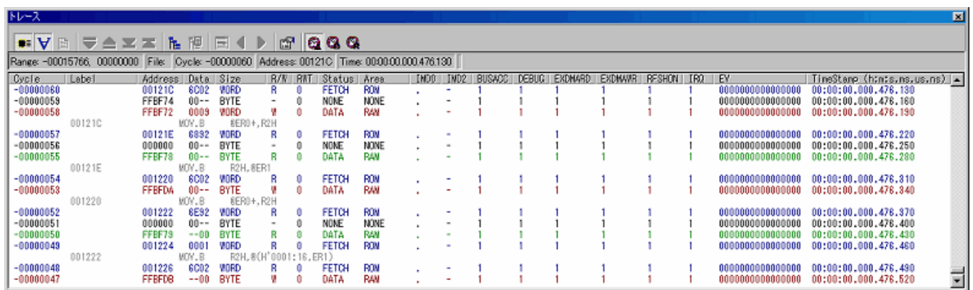
図 5.60 [トレース] ウィンドウ
