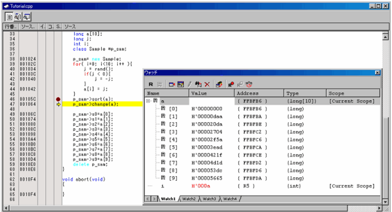
図3. 22 [エディタ]ウィンドウ (ステップアウト)
