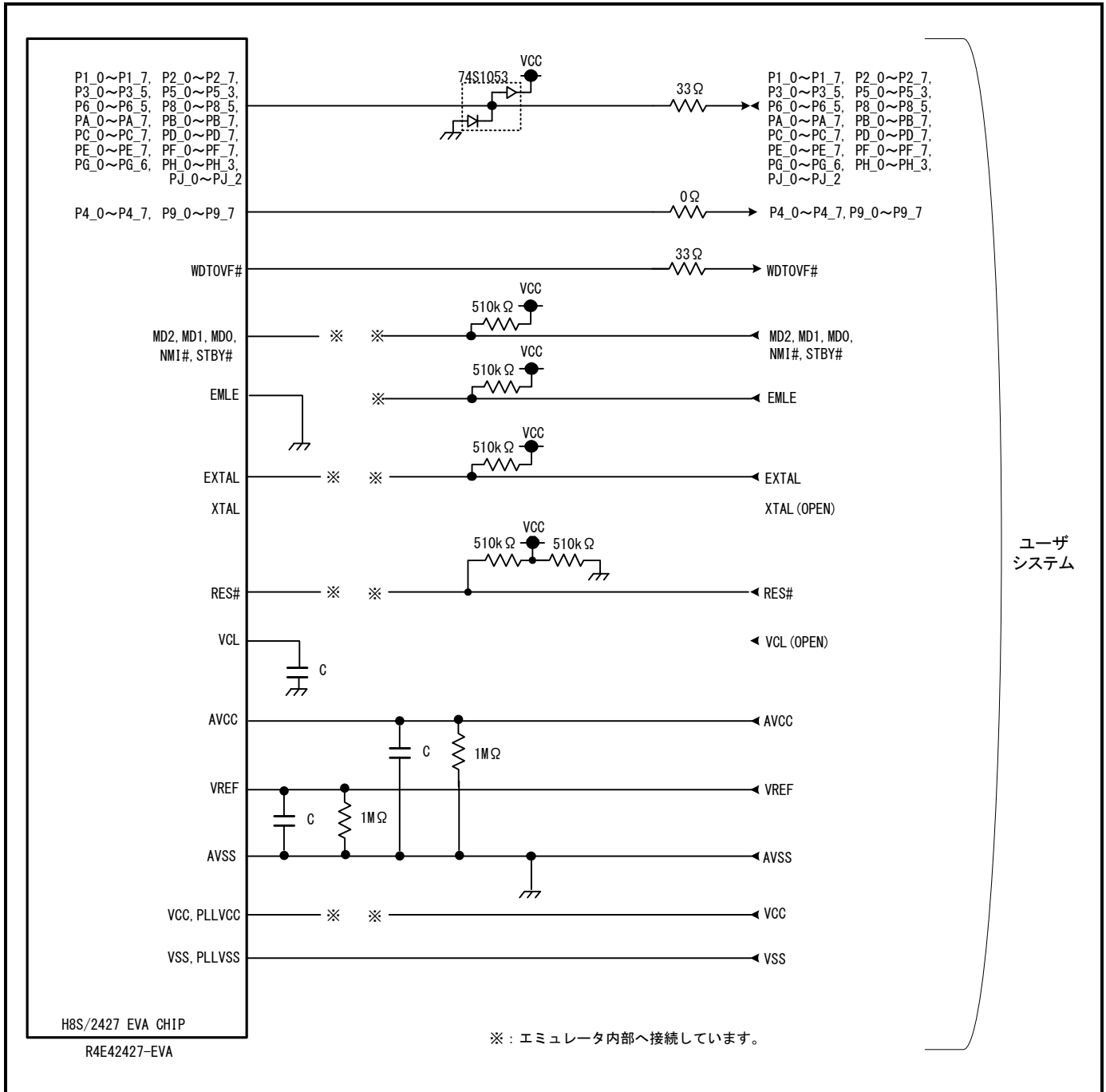
図 7.1 R0E424270MCU00の接続図(一部)
