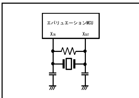
図2.9 エミュレータでは使用できない発振回路
