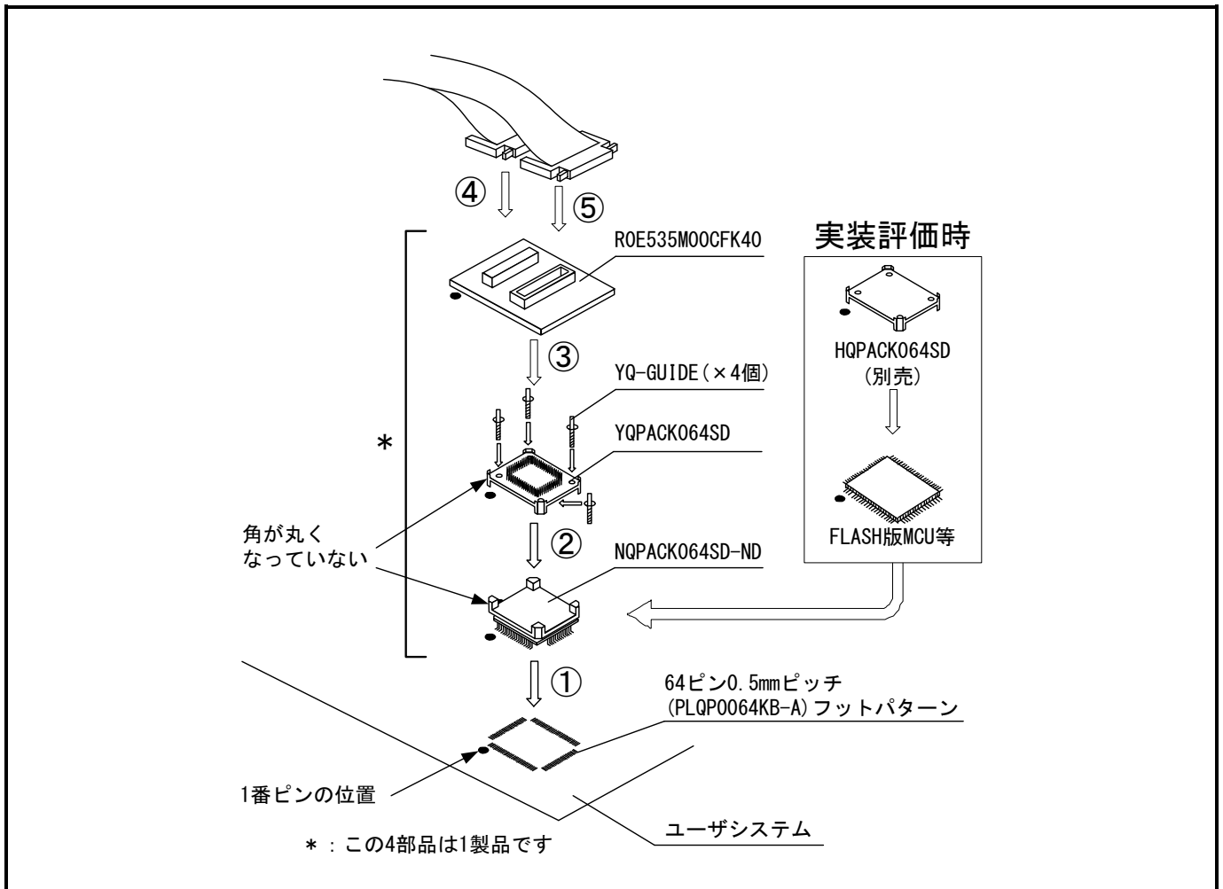
図2.13 64ピン0.5mmピッチフットパターンへの接続
