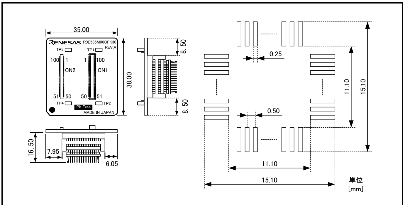
図7.4 R0E535M00CFK30ユーザーシステム接続部の寸法図および参考フットパターン
