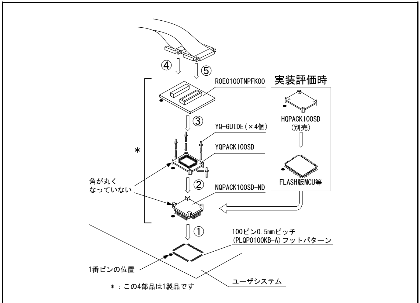
図2.11 100ピン0.5mmピッチフットパターンへの接続
