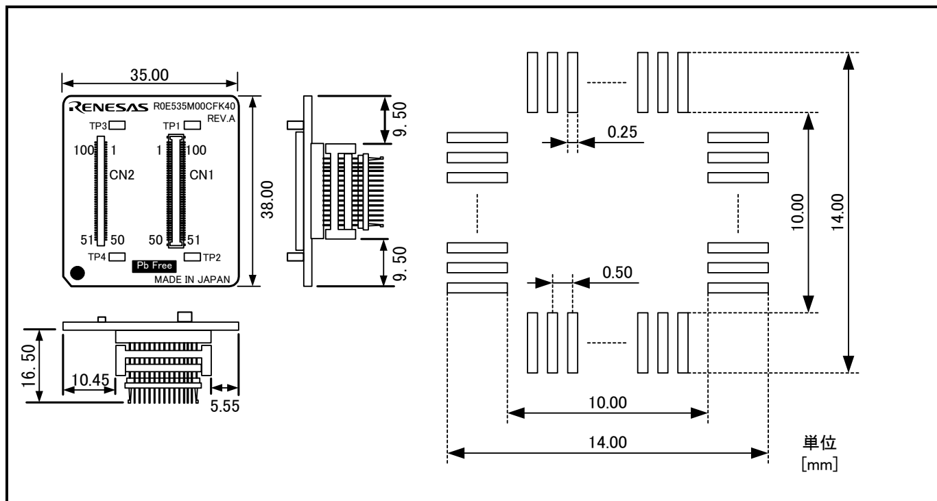
図7.5 R0E535M00CFK40ユーザーシステム接続部の寸法図および参考フットパターン
