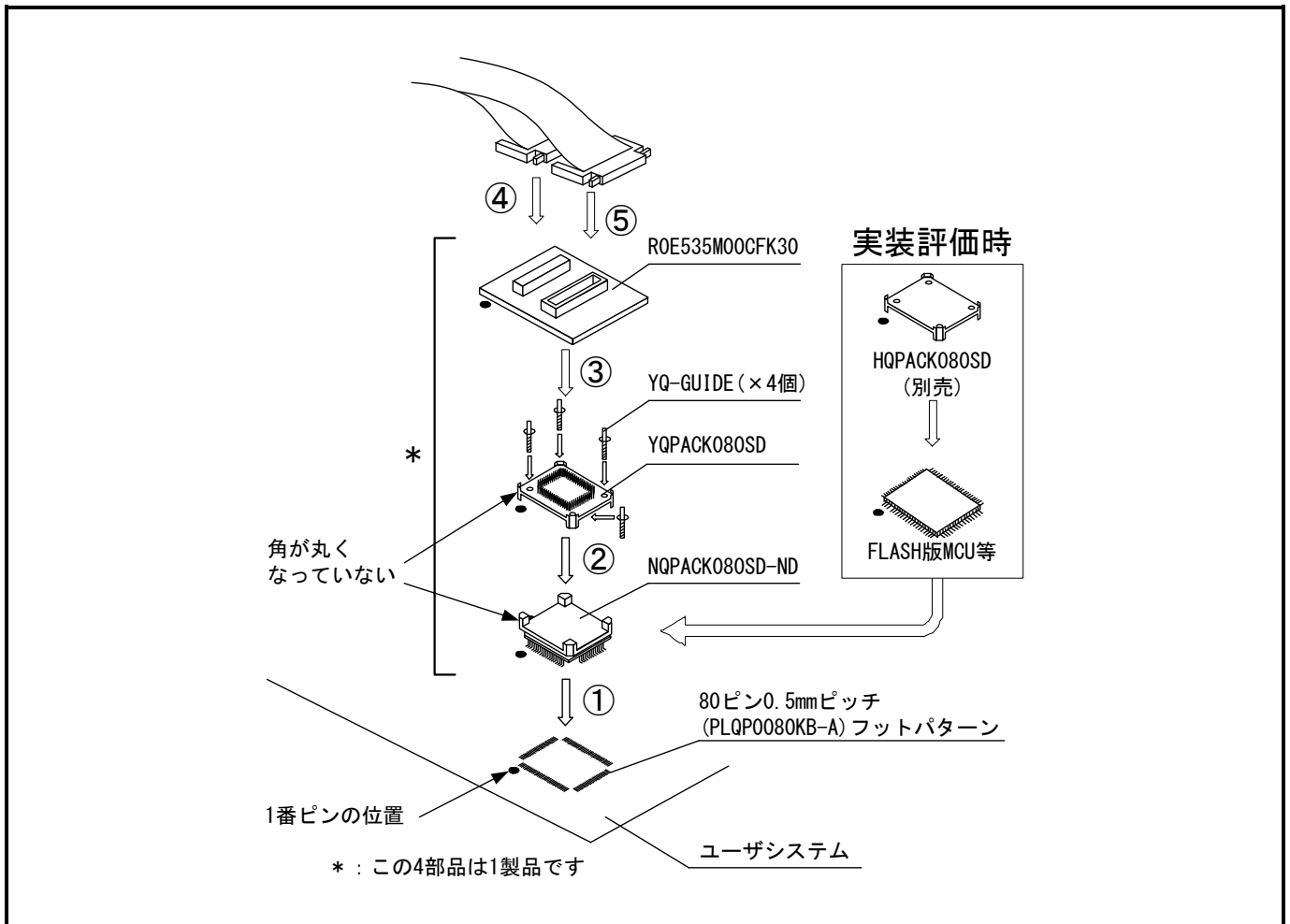
図2.12 80ピン0.5mmピッチフットパターンへの接続
