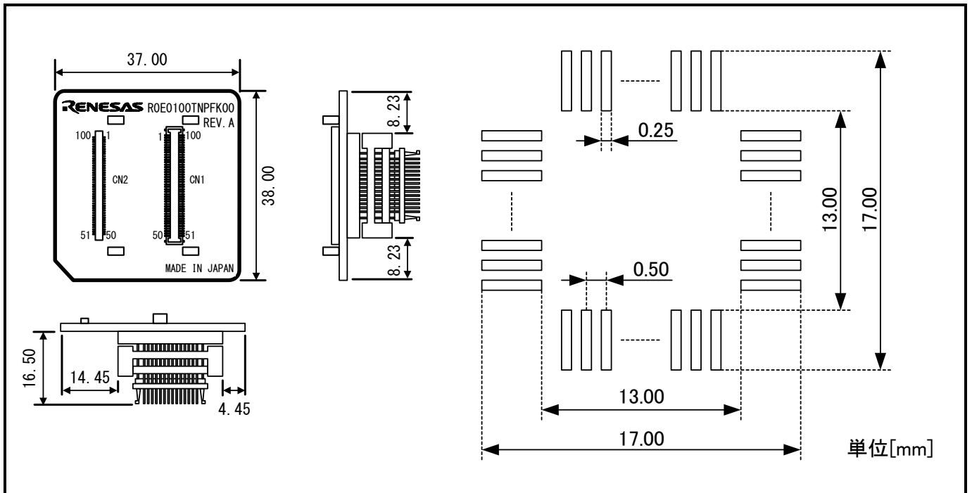
図7.3 R0E0100TNPFK00ユーザーシステム接続部の寸法図および参考フットパターン
