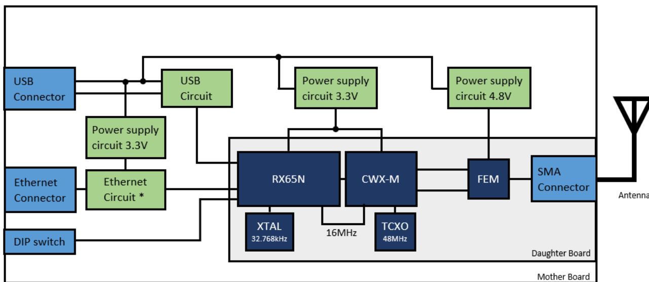
図 1-1 : ブロック図
