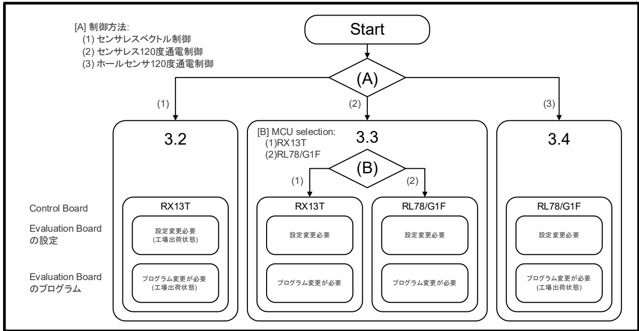
Figure 3-2 RAA306012 RSSK のモータ評価設定
