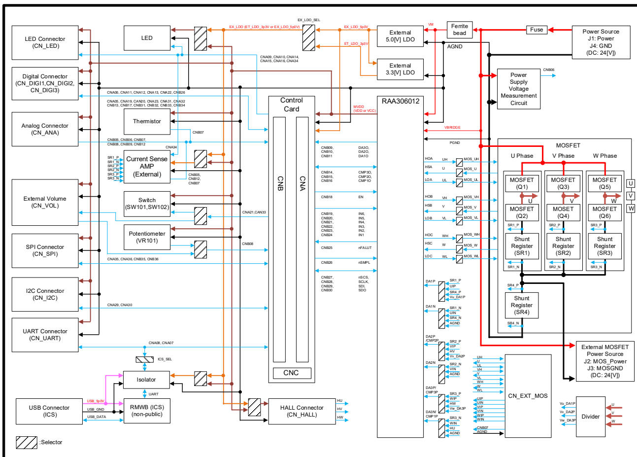
Figure 2-2 ブロック図
