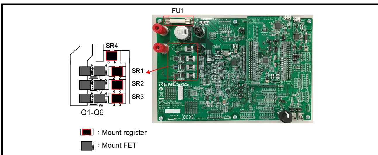
Figure 4-14 部品変更箇所 (他モータ使用時)
