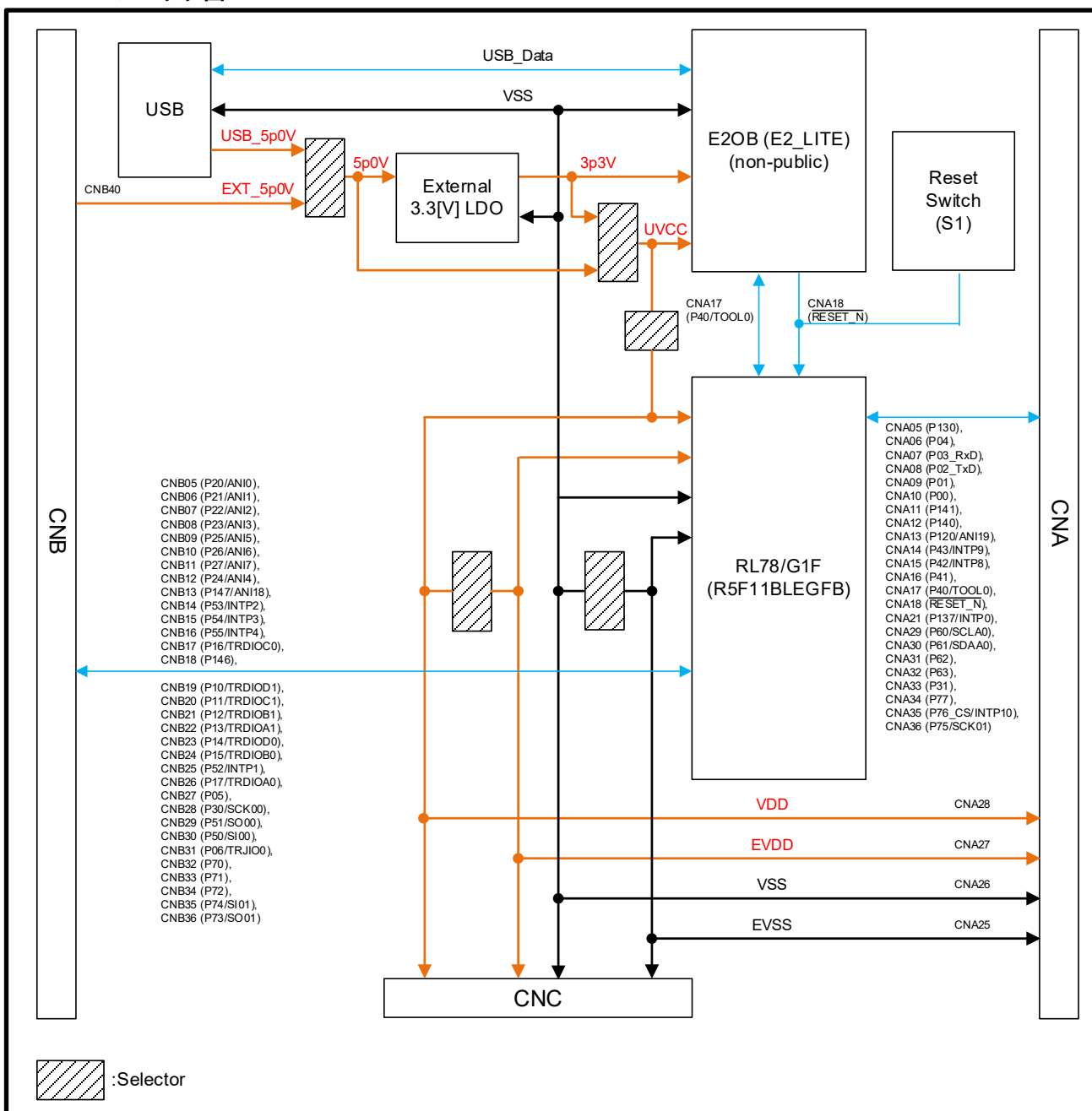
Figure 2-9 ブロック図
