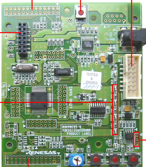
LCD モジュール コネクタ
