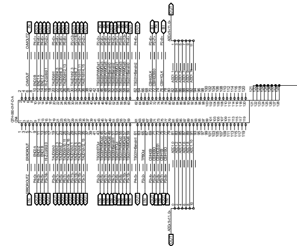
CONNECTOR4
