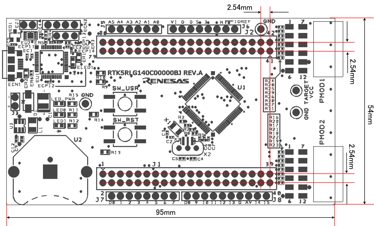
図 3-1: 部品配置図
