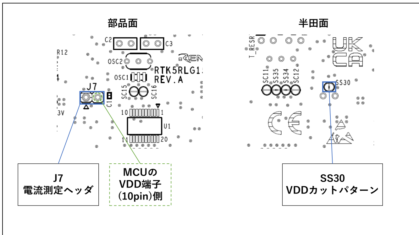
図 5-9: 電流測定ヘッド および VDD カットパターン位置
