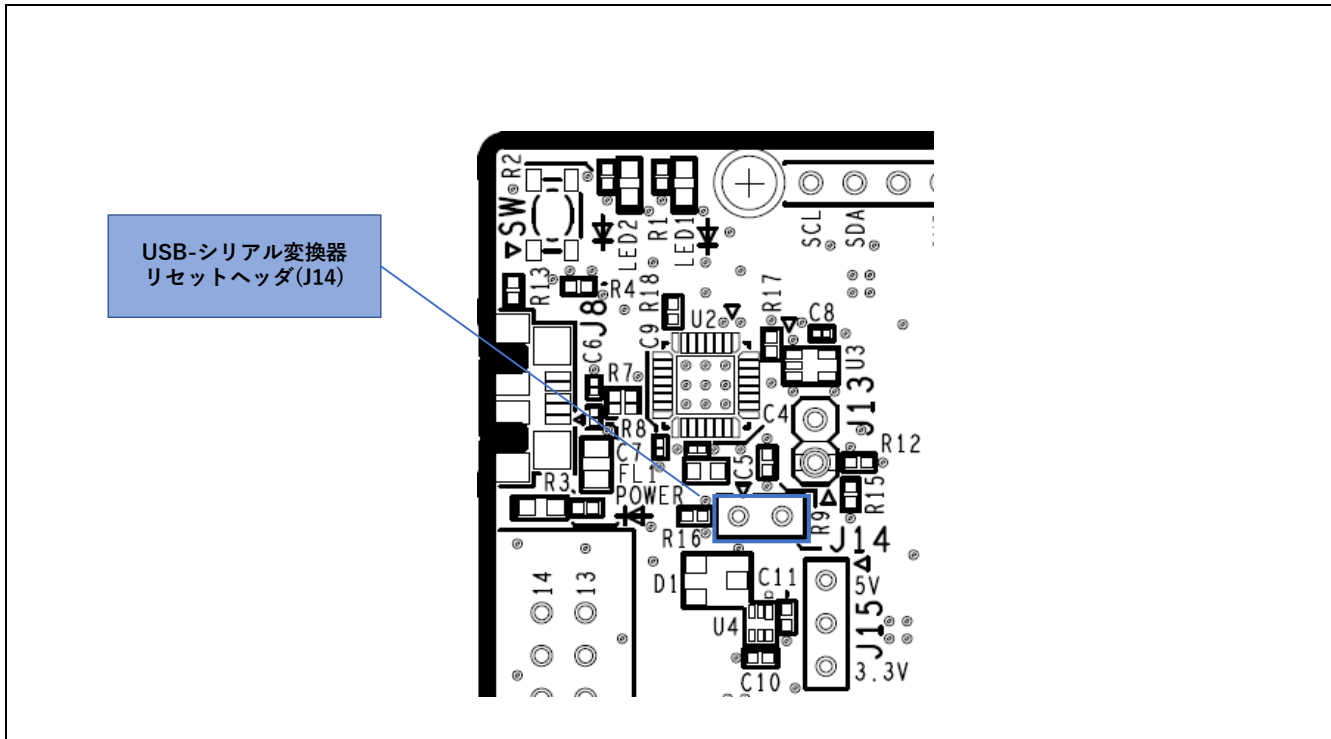
図 5-3: USB-シリアル変換器リセットヘッダ位置(部品面)
