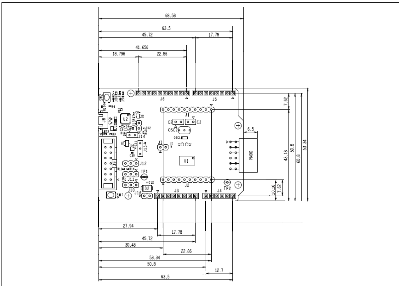
図 3-2: 寸法図
