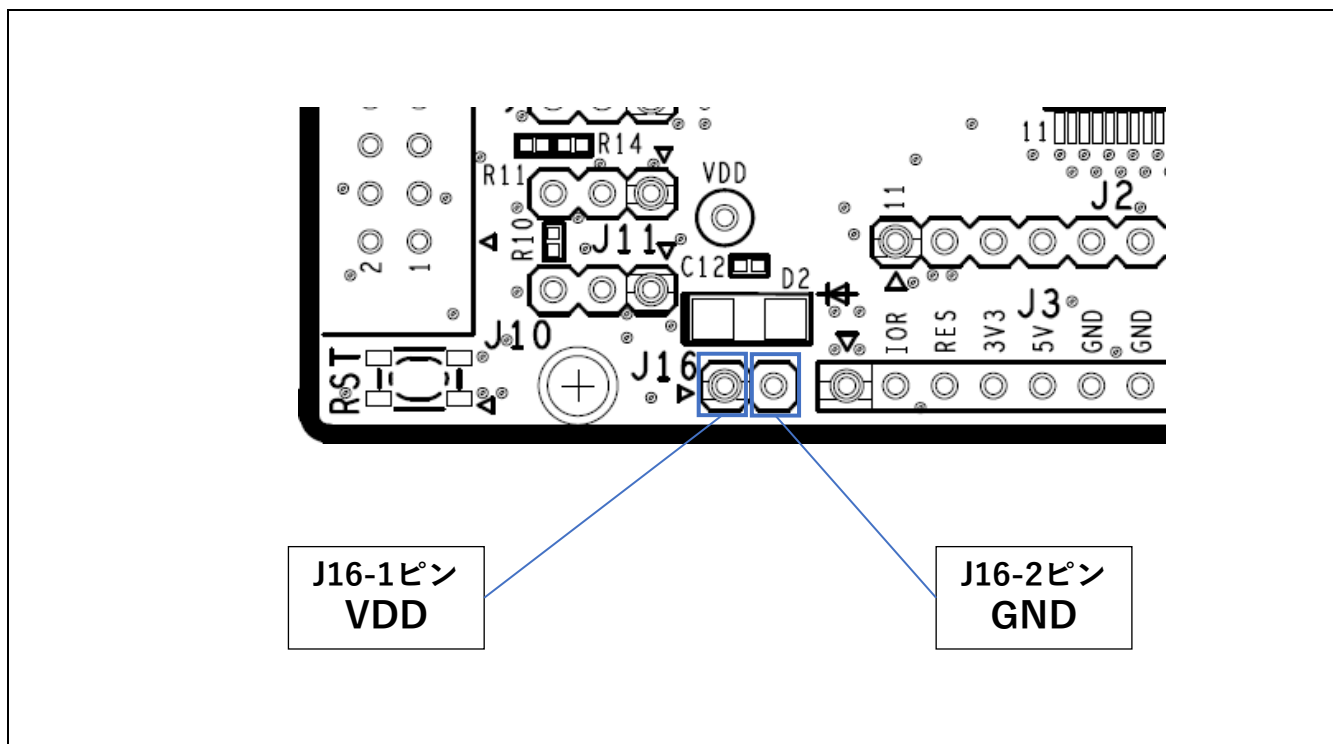
図 5-8: 外部電源供給接続先位置(部品面)
