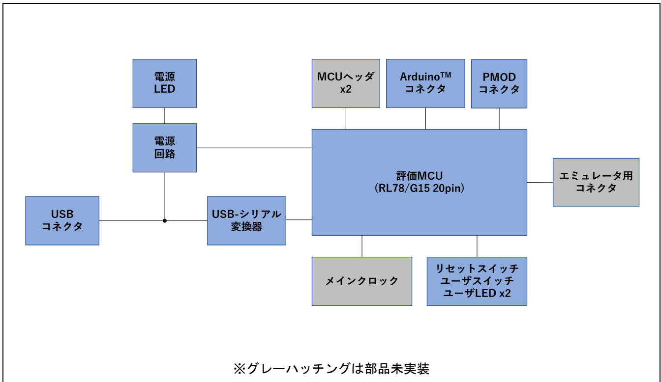
図 1-1:ブロック図
