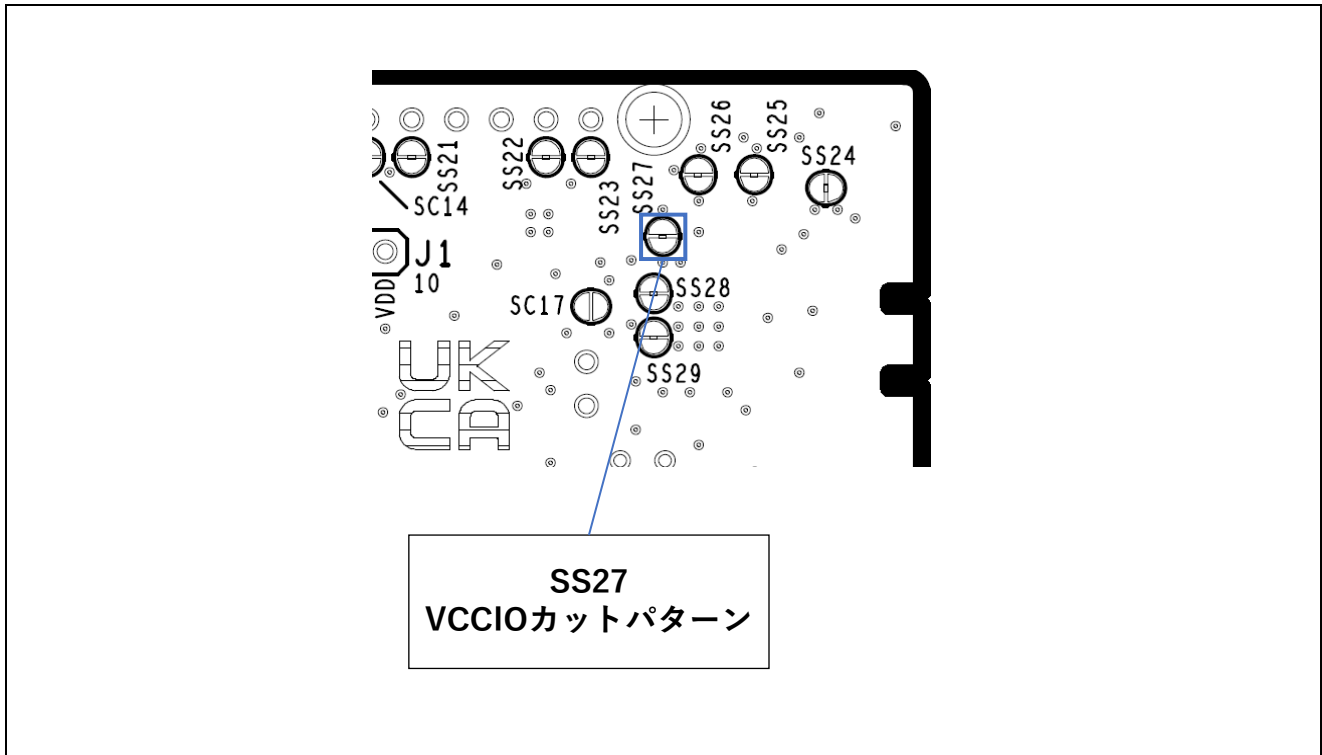
図 5-11: VCCIO カットパターン位置
