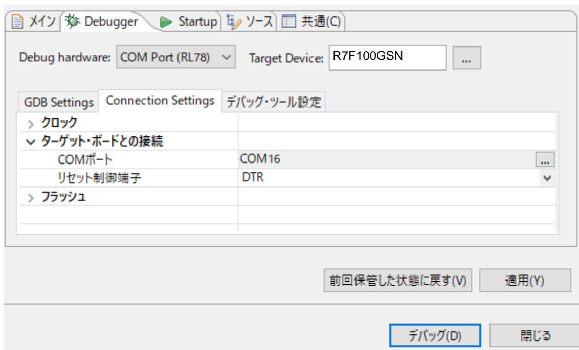
図 8-25: e 2 studio の設定
