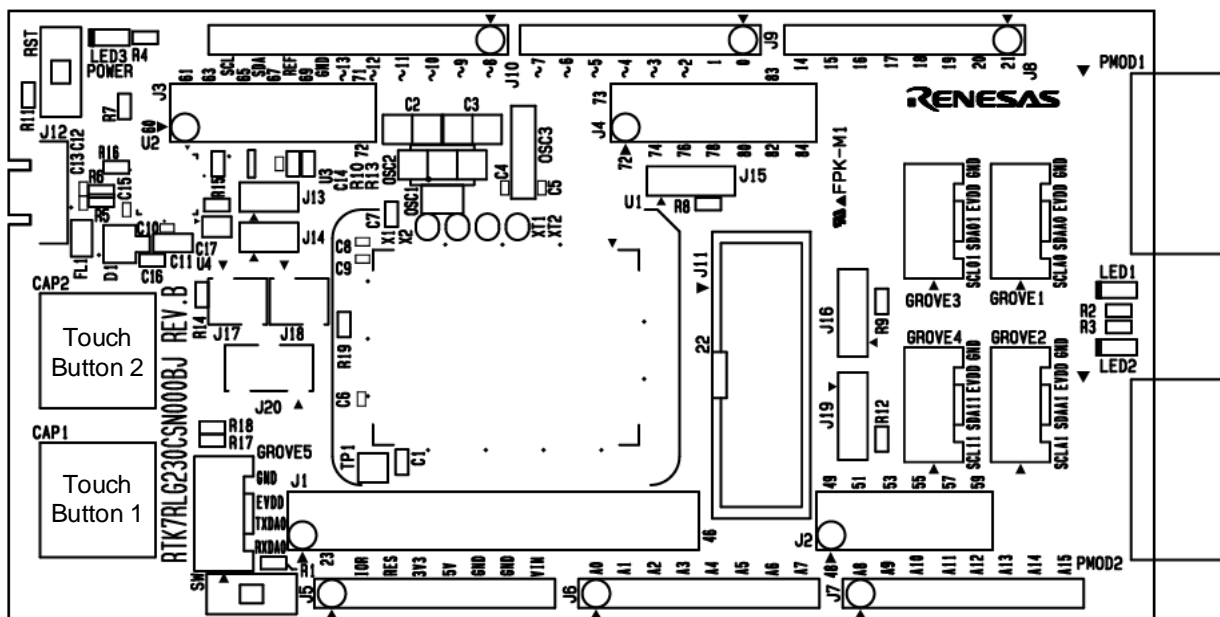
図 8-3: 部品配置図
