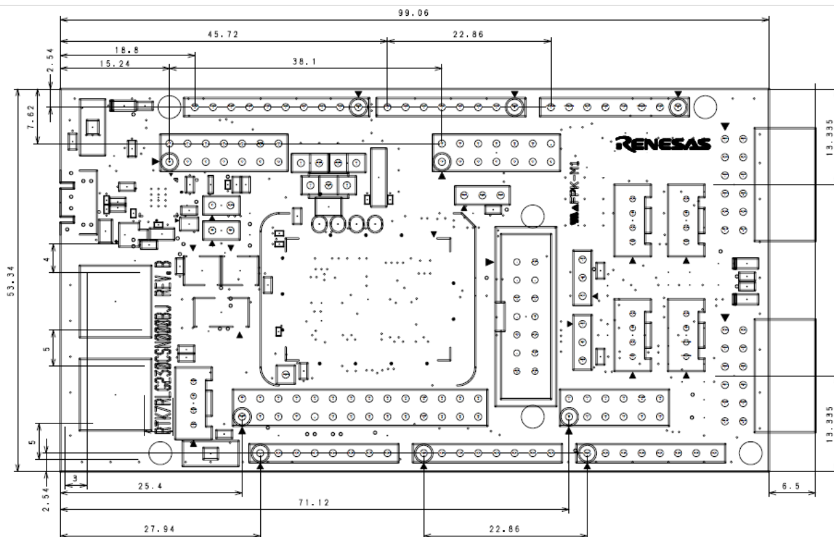
図 8-4: 寸法図
