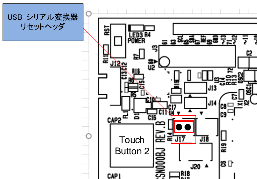
図 8-9: USB-シリアル変換器リセットヘッダ位置(部品面)
