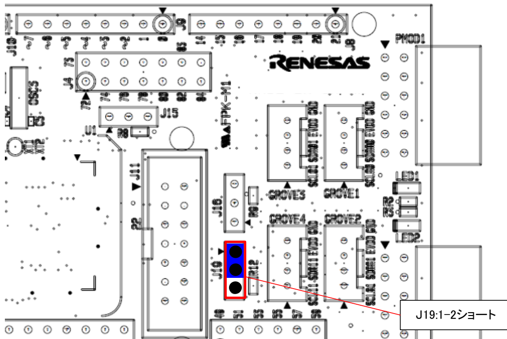
図 8-24 : COM port デバッグ使用時設定(部品面)
