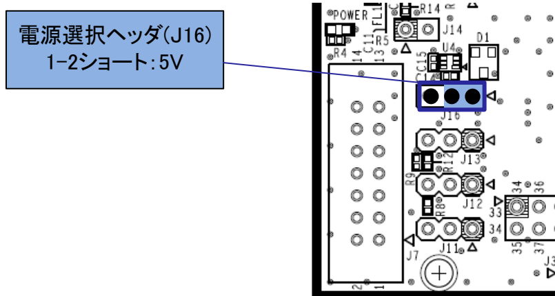
図 5-5: 5V 使用時のヘッダ設定(部品面)
