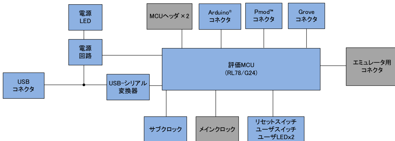
図 1-1: ブロック図
