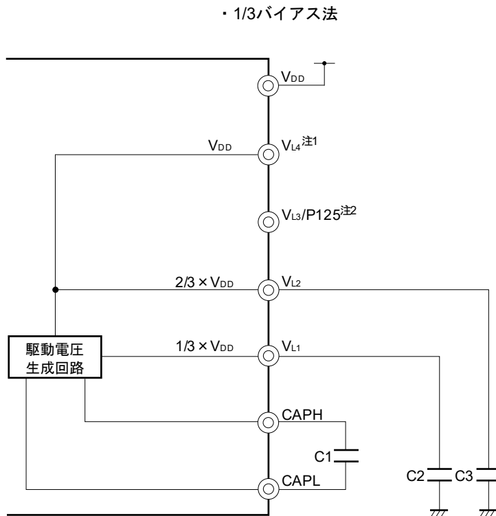
図16-23 LCD駆動用電源の接続例（容量分割方式）
