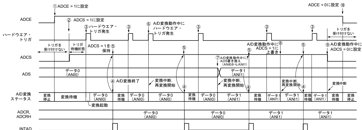
図12-20 ハードウェア・トリガ・ノーウエイト・モード（ワンショット変換モード）動作タイミング例
