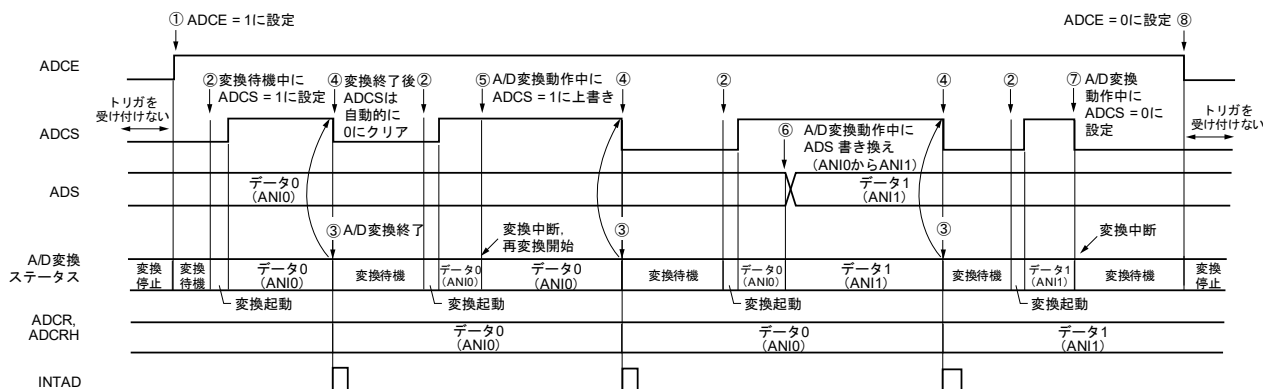
図12-18 ソフトウェア・トリガ・モード（ワンショット変換モード）動作タイミング例
