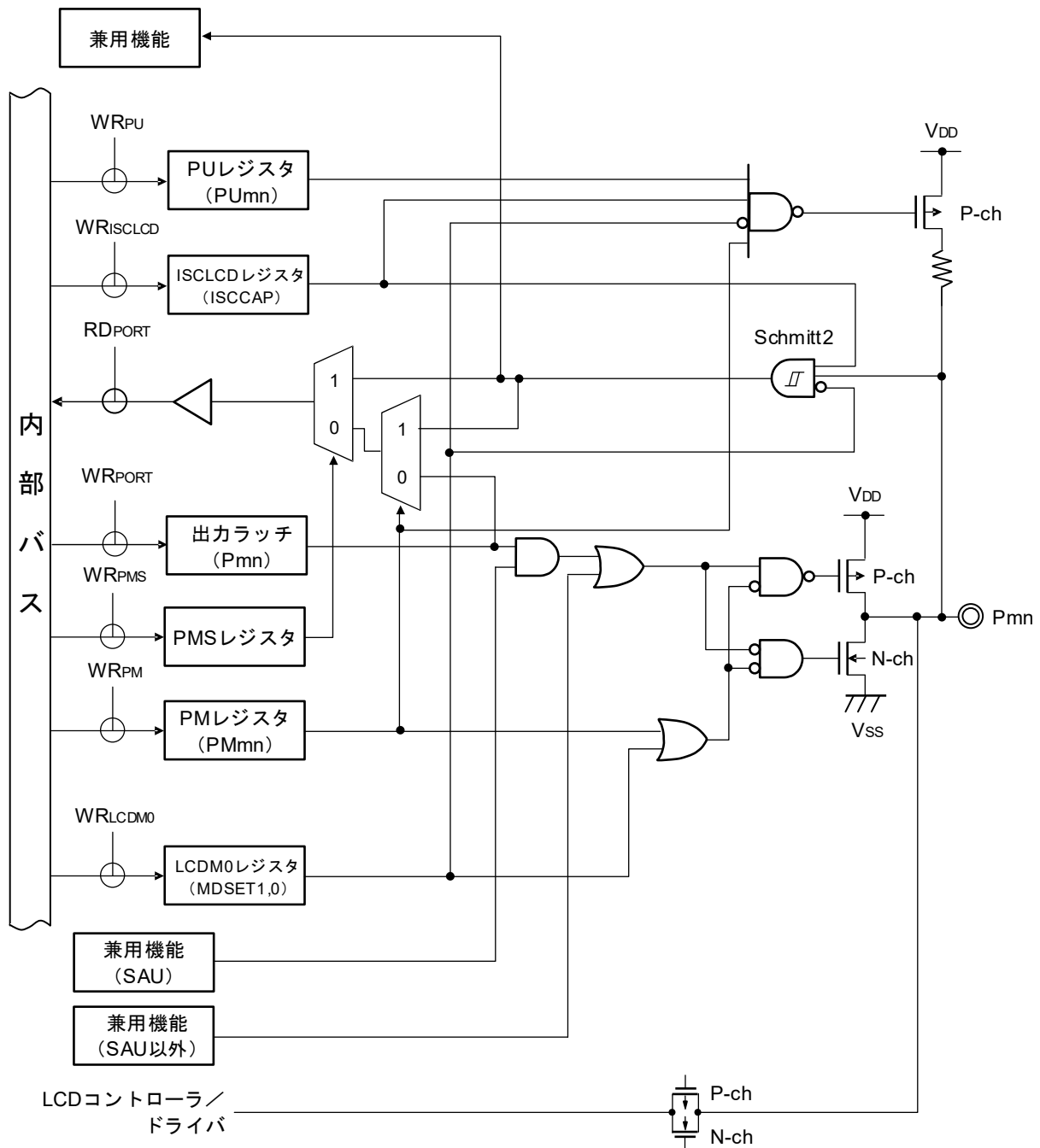
図2-7 端子タイプ 7-5-5 の端子ブロック図
