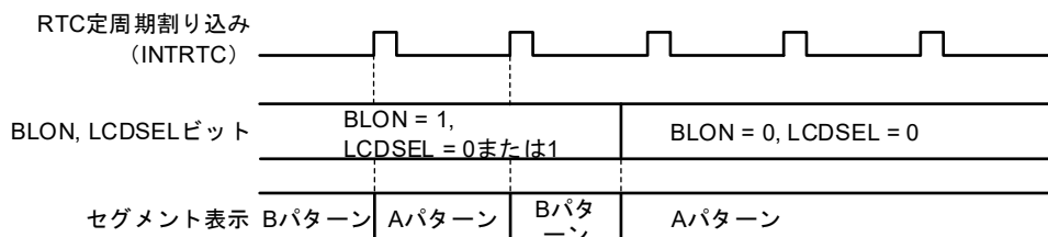
図16-16 点滅表示からAパターン表示への切り替え動作
