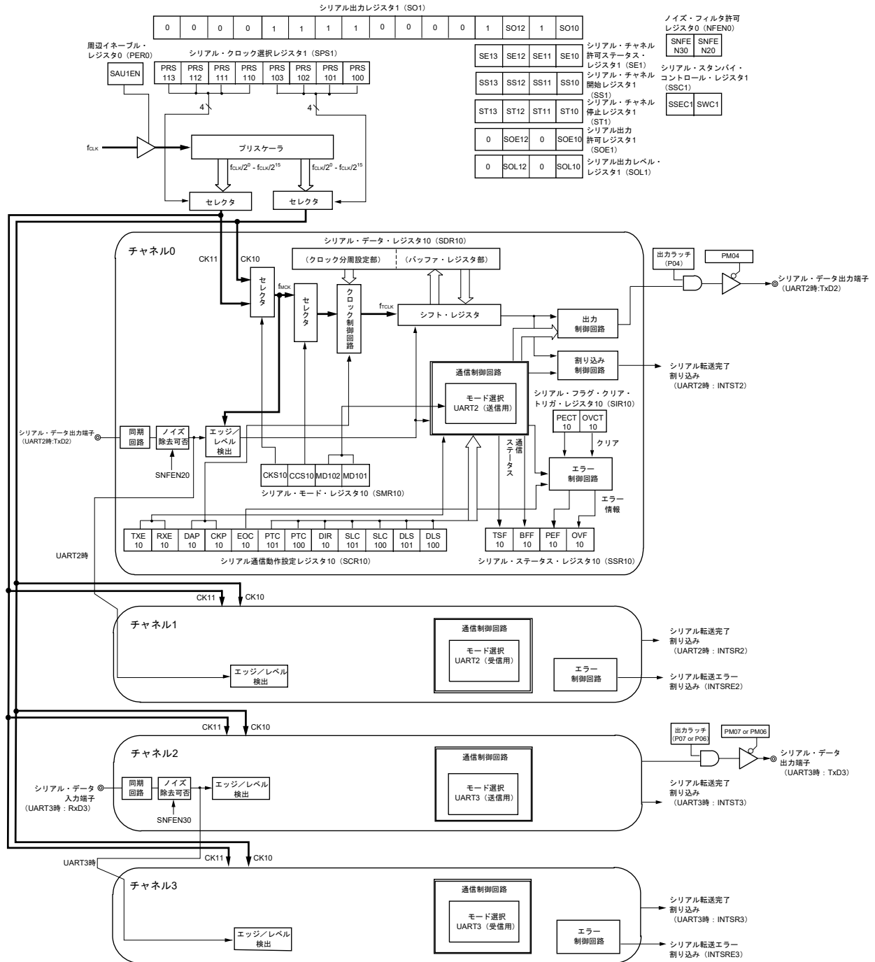
図14-2 シリアル・アレイ・ユニット1のブロック図 (80ピン製品)
