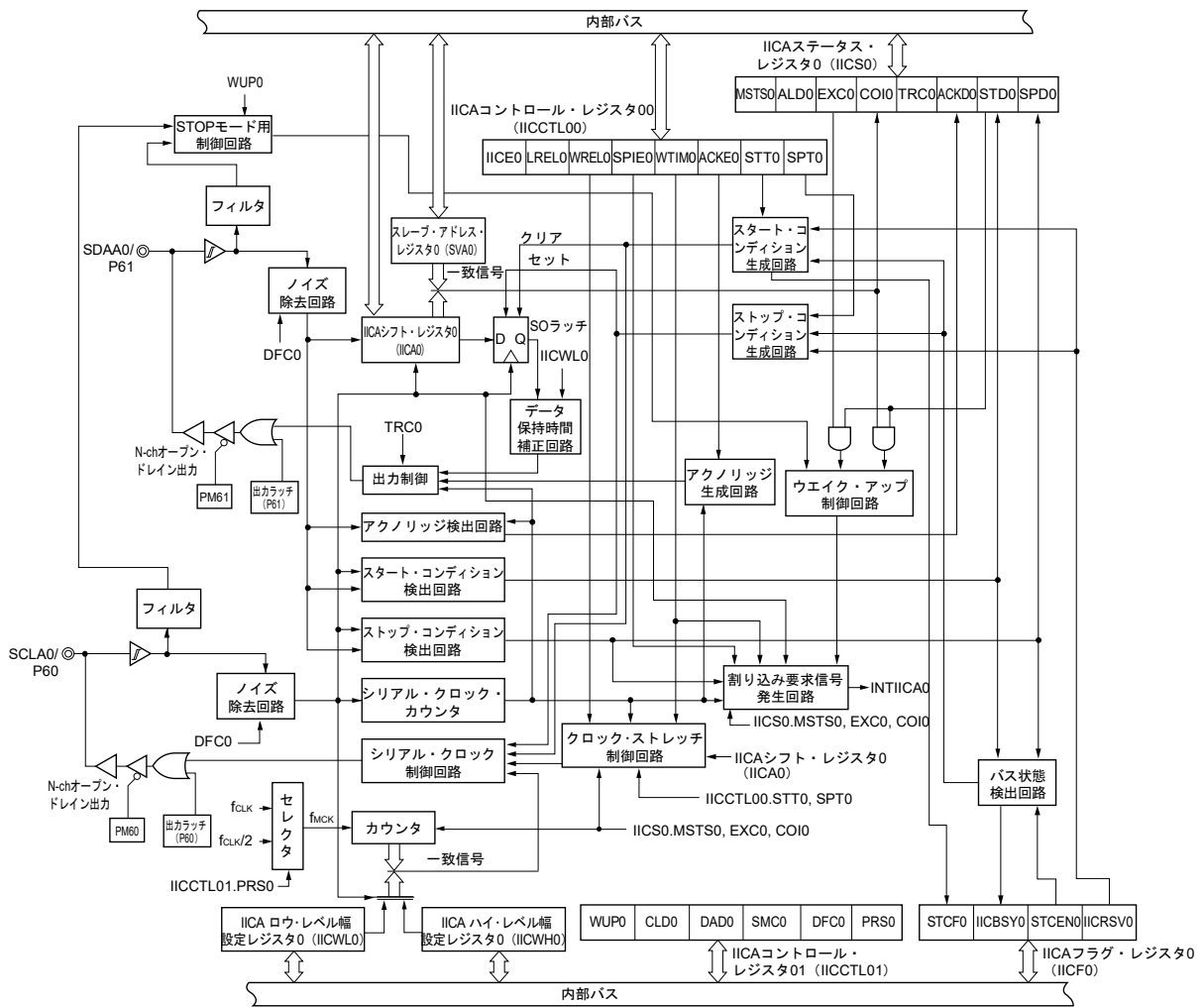
図15-1 シリアル・インタフェースIICA0のブロック図
