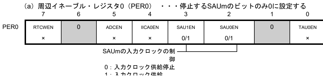
図14-23 ユニット単位で動作停止とする場合の周辺イネーブル・レジスタ0 (PER0) の設定
