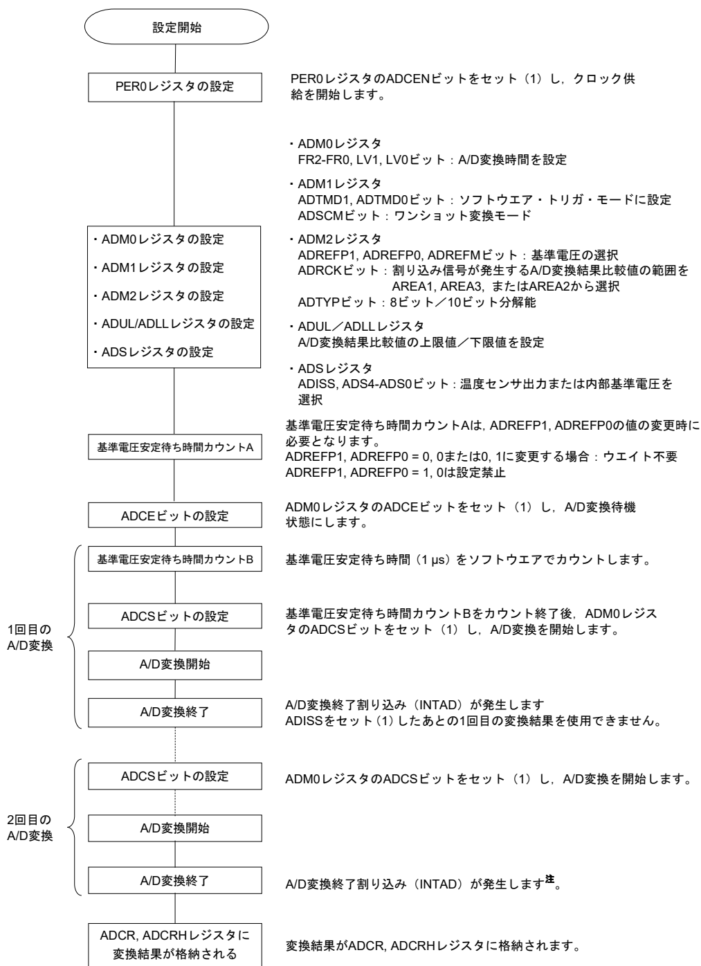
図12-26 温度センサ使用時の設定
