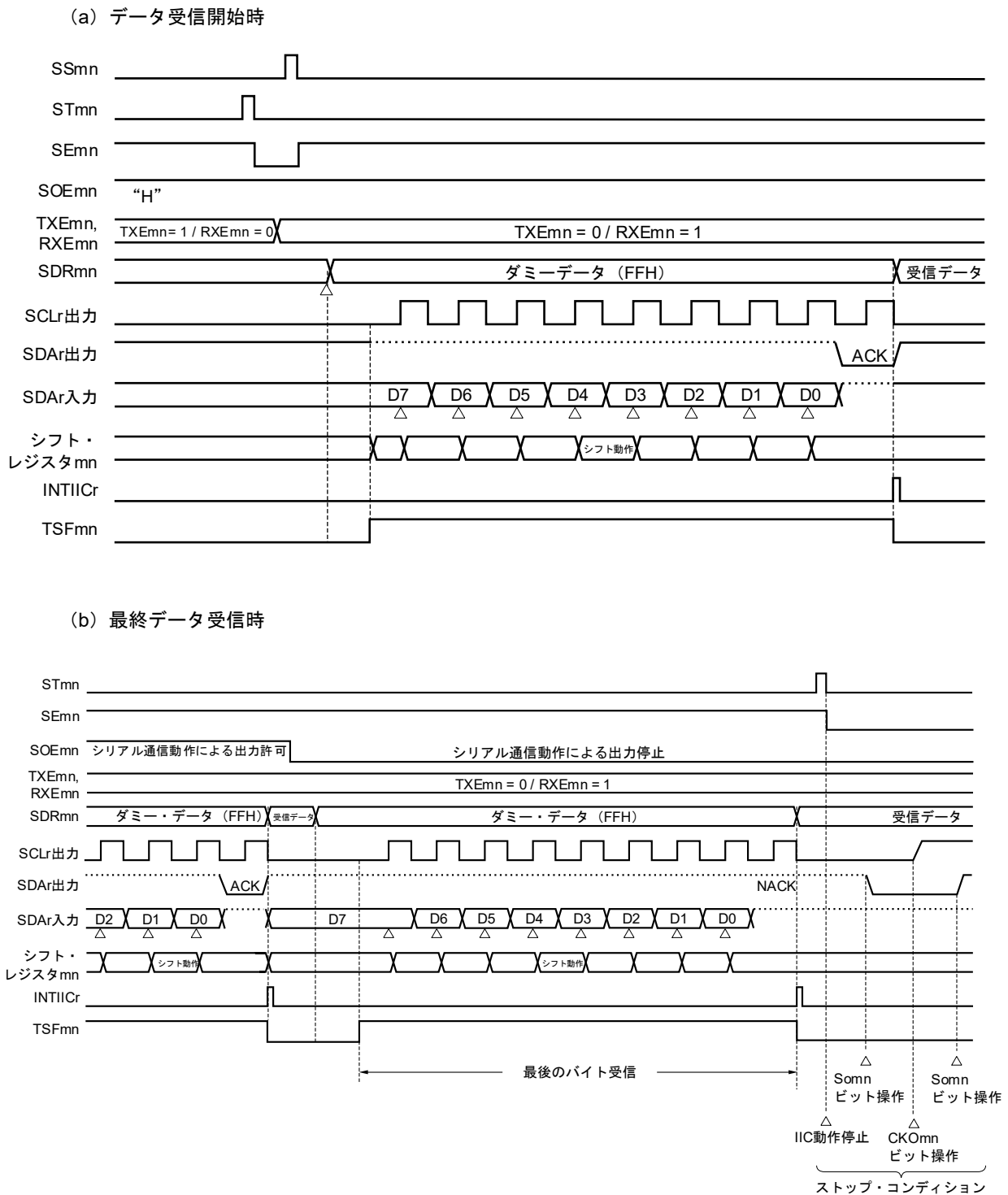
図14-111 データ受信のタイミング・チャート
