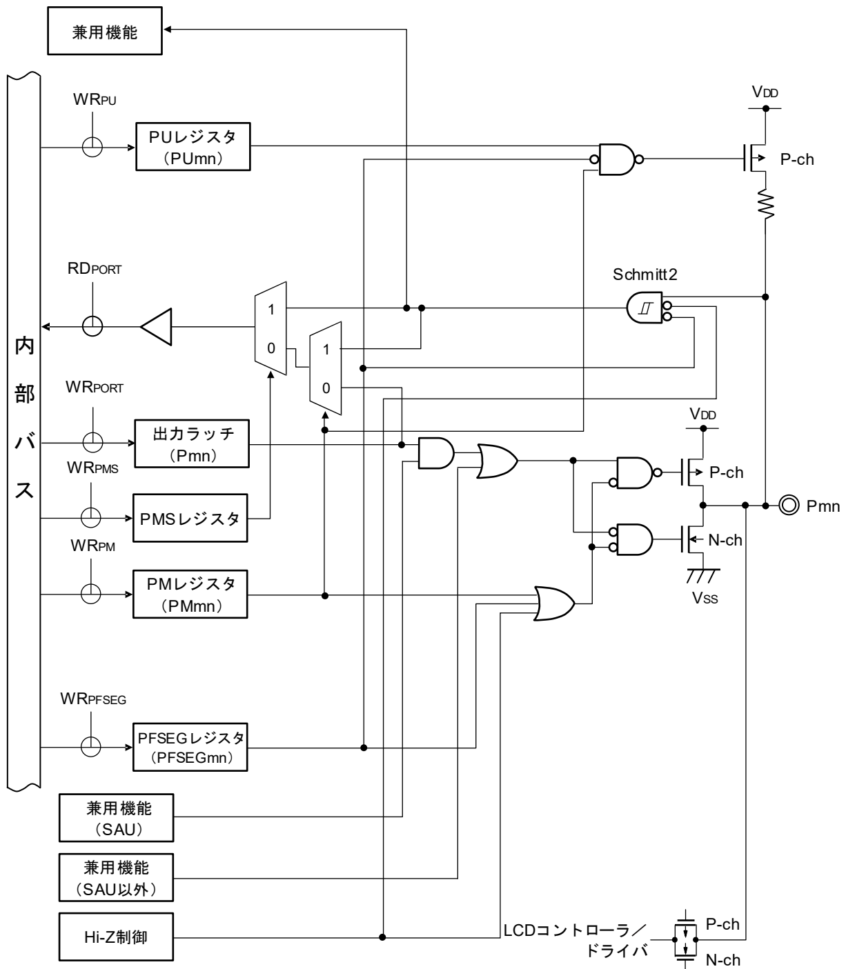
図2-10 端子タイプ 7-5-16 の端子ブロック図
