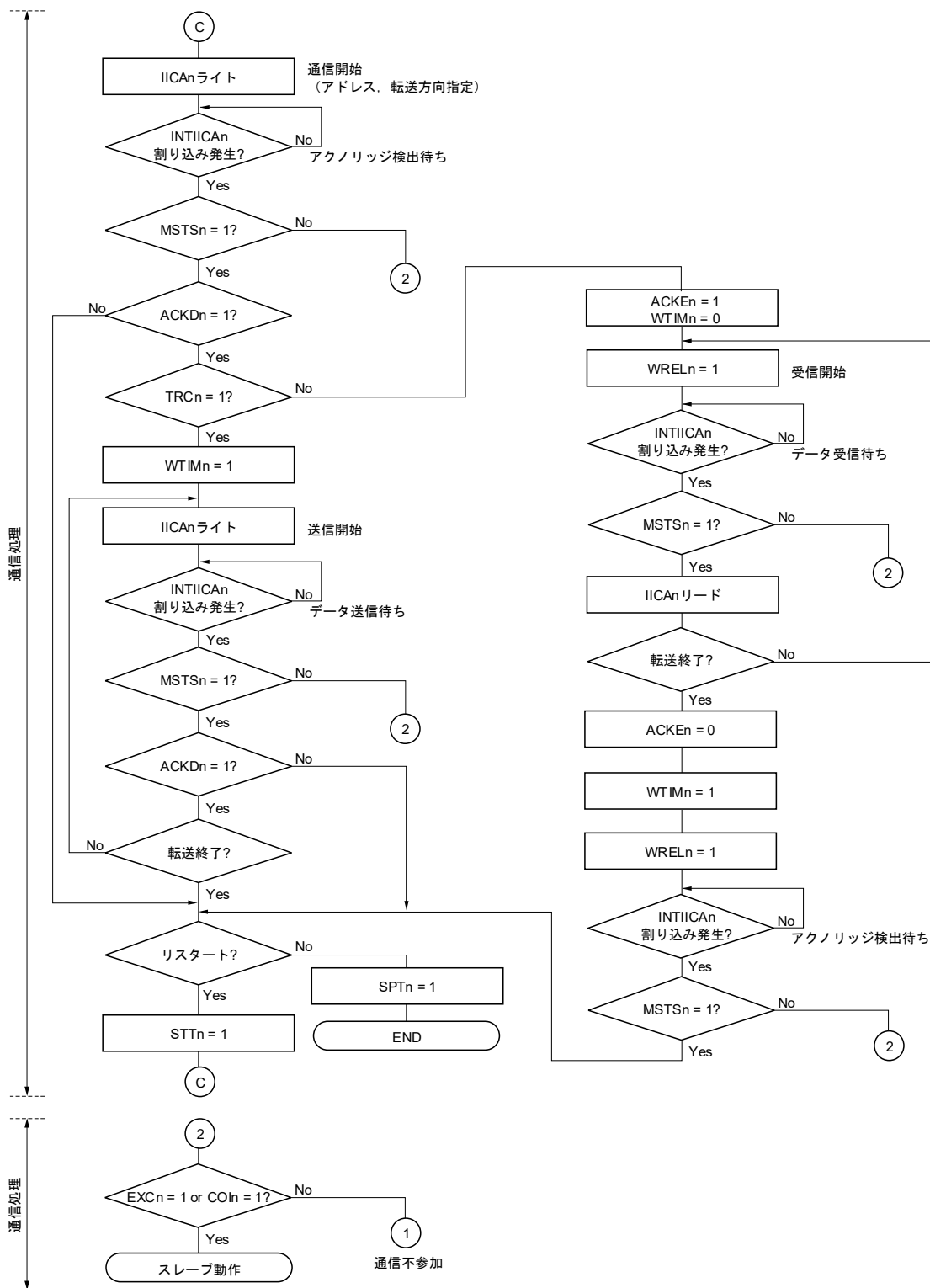
図15-29 マルチマスタ・システムでのマスタ動作 (3/3)
