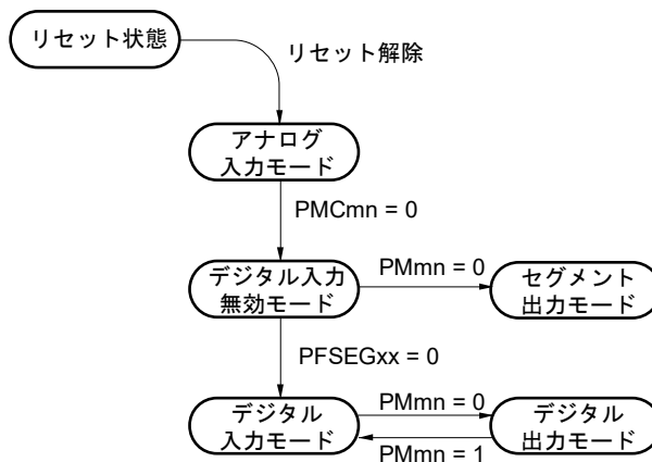
図4-13 ANLxx/SEGxx/ポート端子機能の状態遷移図
