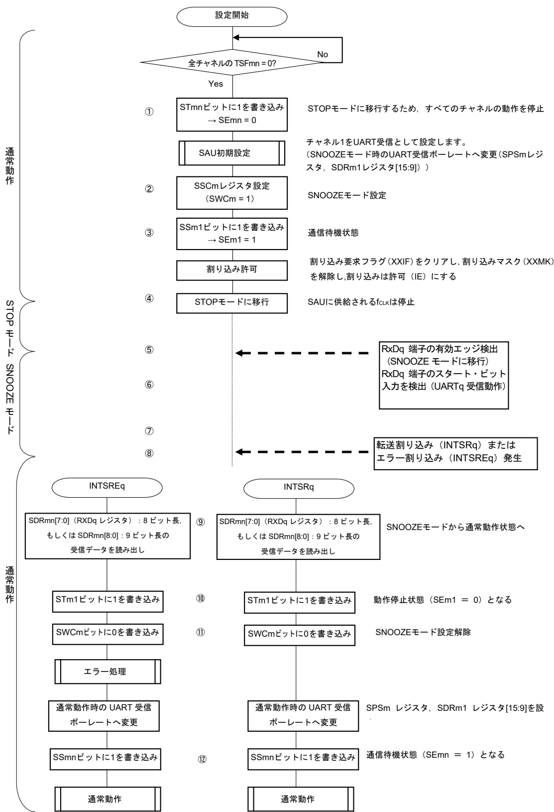
図14-92 SNOOZEモード動作 (EOCm1 = 0, SSECm = 0/1もしくはEOCm1 = 1, SSECm = 0) 時の
