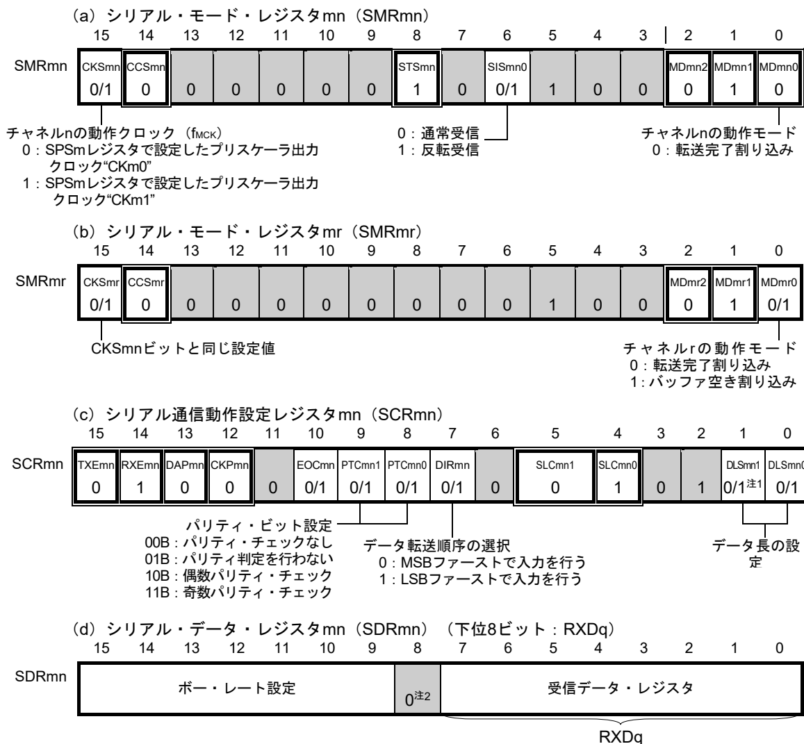
図14-84 UART (UART0-UART3) のUART受信時のレジスタ設定内容例 (80ピン製品) (1/2)
