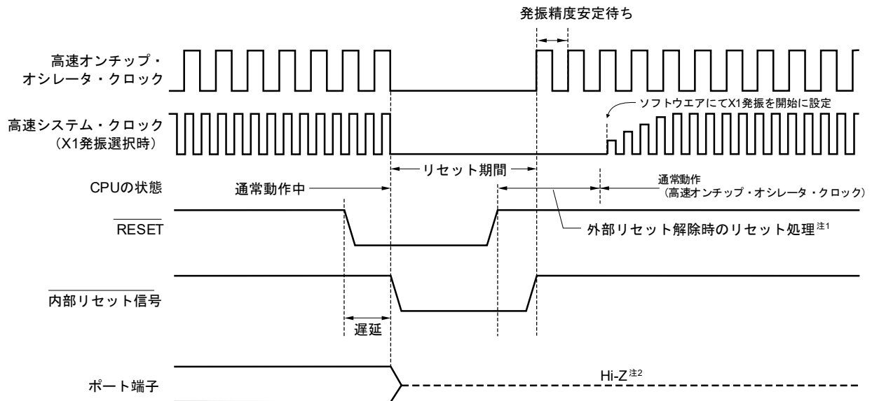
図22-2 \overline{\text{RESET}} 入力によるリセット・タイミング
