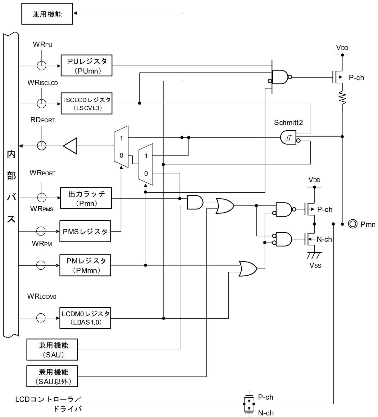
図2-8 端子タイプ 7-5-6 の端子ブロック図
