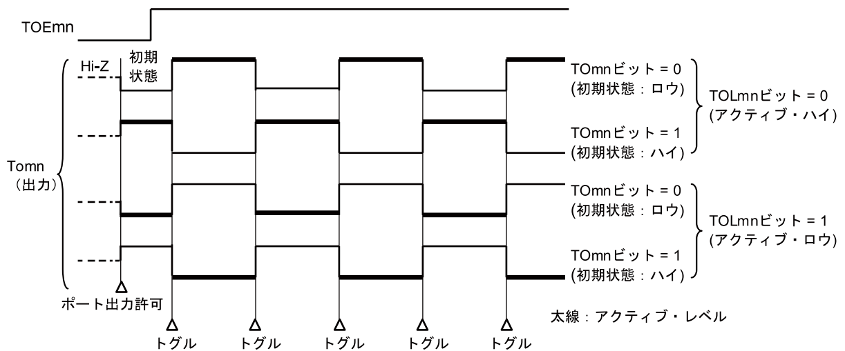
図6-34 トグル出力時 (TOMmn = 0) のTOmn端子出力状態
