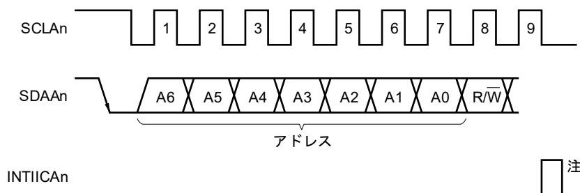
図15-16 アドレス
