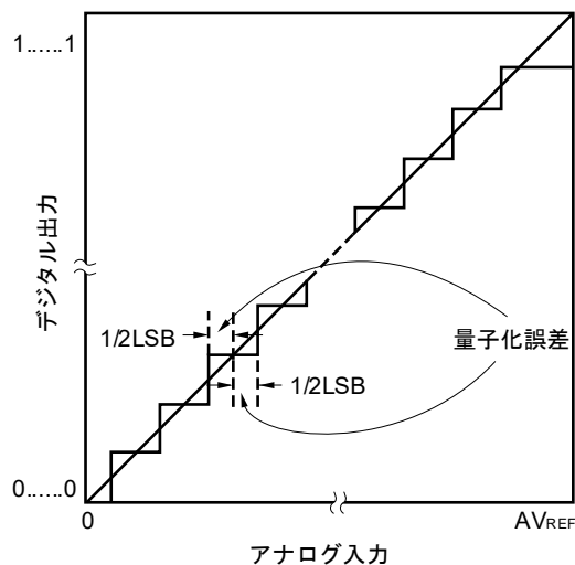
図12-33 量子化誤差
