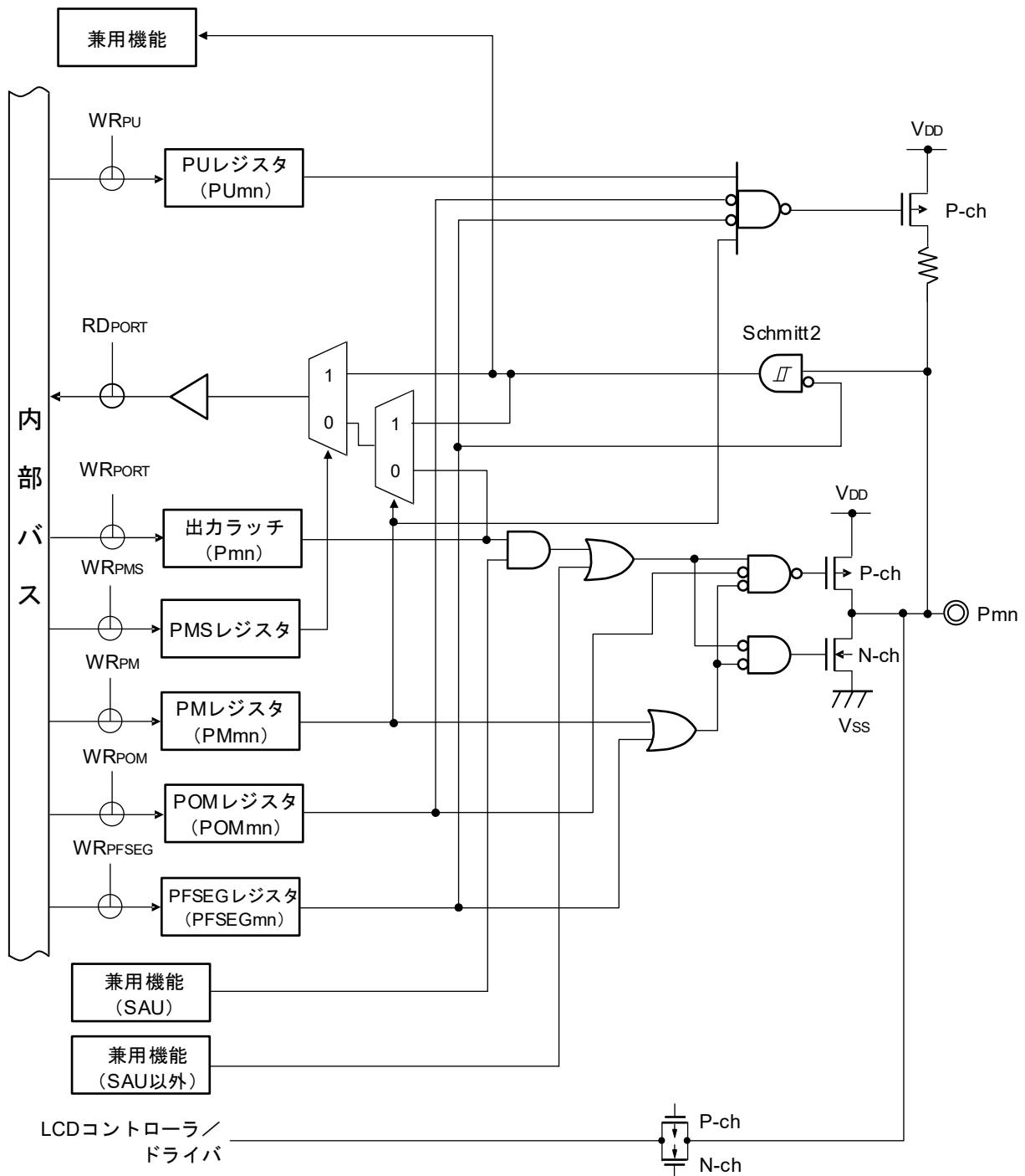
図2-9 端子タイプ 7-5-10 の端子ブロック図
