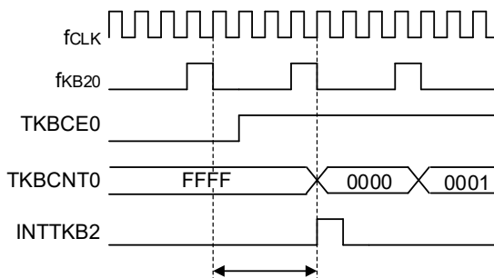
図7-35 動作開始のタイミング図 (TKBCE0を“0”から“1”に変更した場合)
