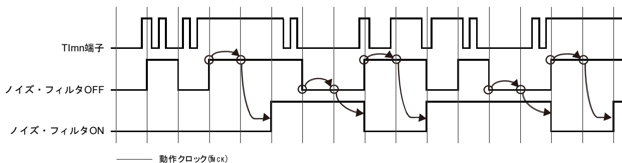
図6-42 Tlmn入力端子に対するノイズ・フィルタON/OFFによるサンプリング波形
