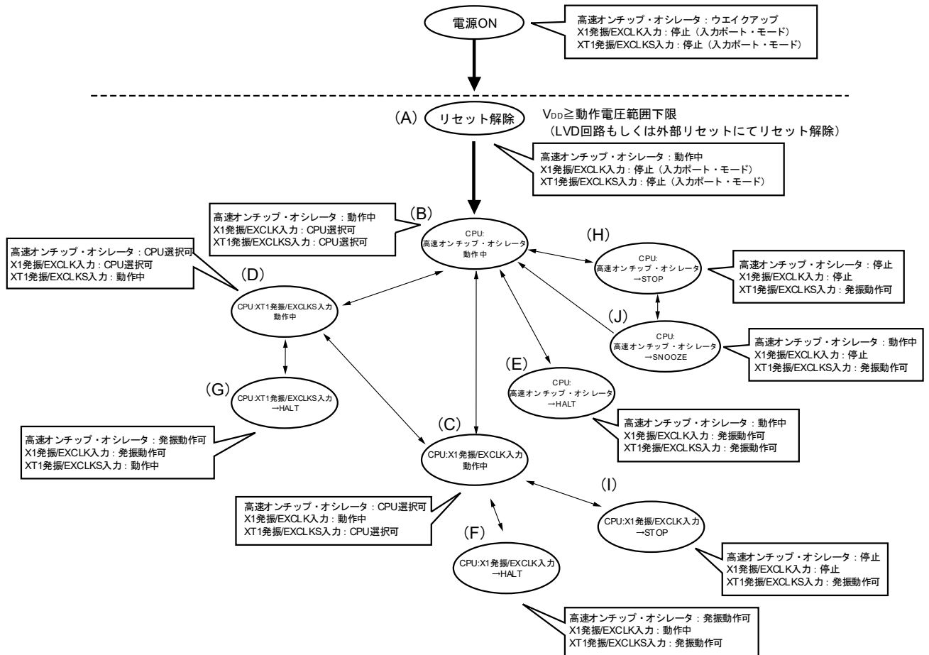
図5-16 CPUクロック状態移行図
