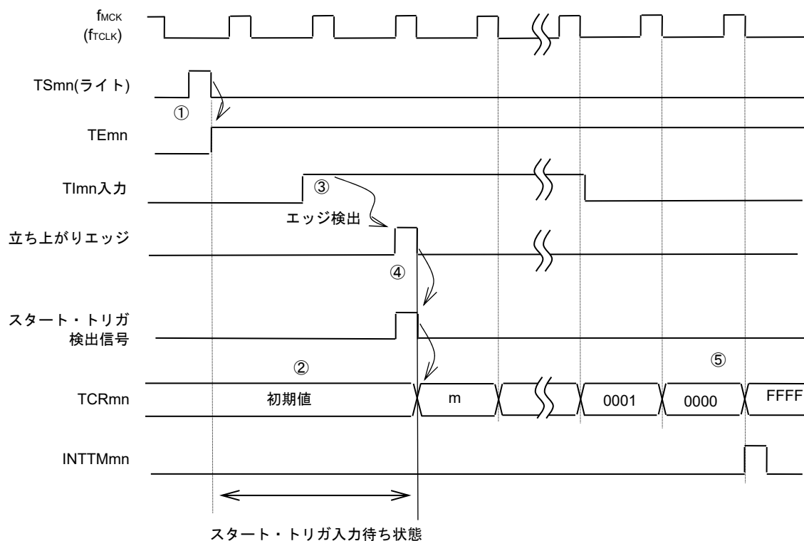
図6-30 動作タイミング (ワンカウント・モード)
