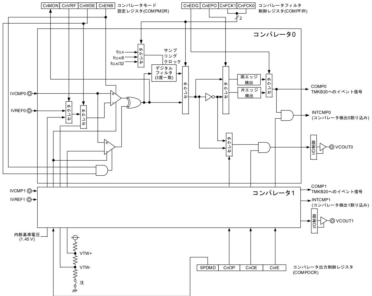
図13-1 コンパレータのブロック図
