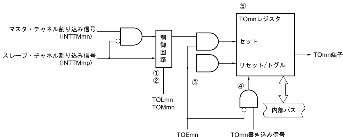
図6-32 出力回路構成図
