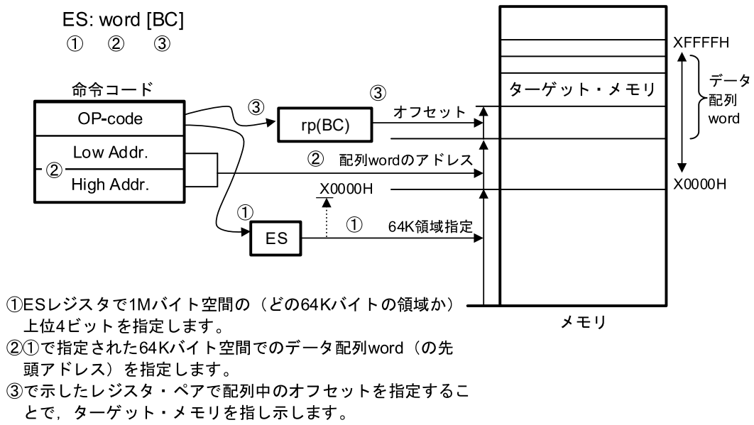
図3-34 ES:word[BC]の例
