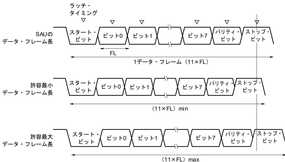
図14-95 受信時の許容ポー・レート範囲 (1データ・フレーム長 = 11ビットの場合)
