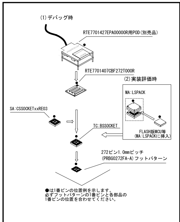
図2 RTE7701407CBF272T000Rの用途
