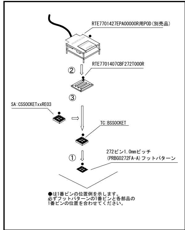
図3 RTE7701407CBF272T000R装着手順
