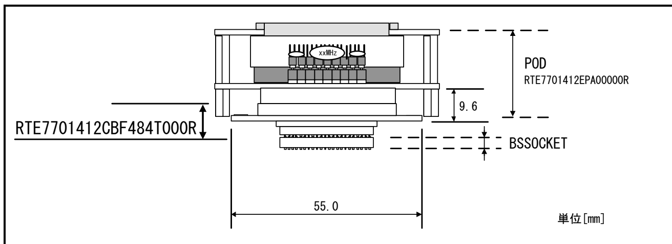
図4 ソケット組立図 (RTE7701412EPA00000Rの場合)
