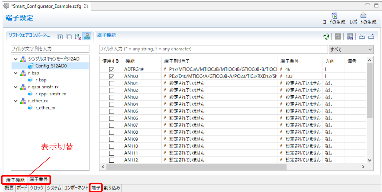
図 4-50 端子ページ（端子機能）
