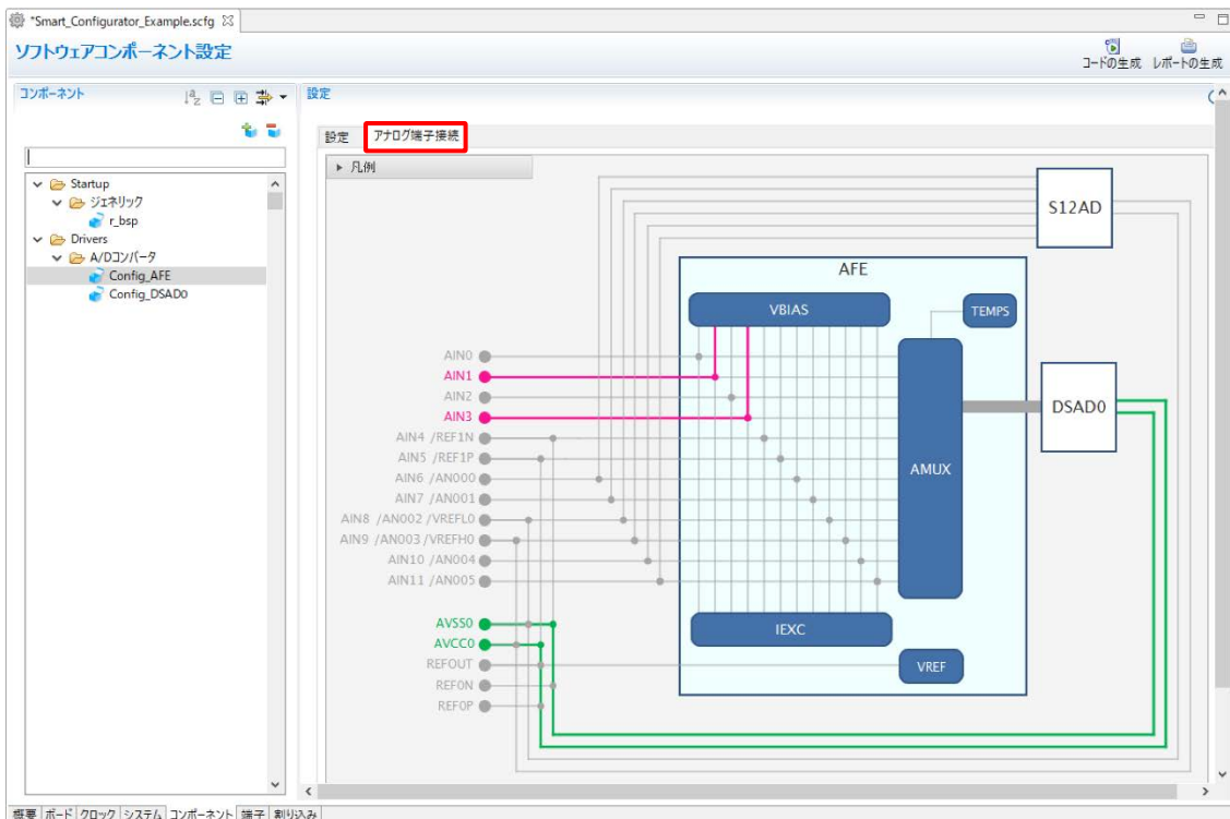
図 4-38 AFE マルチプレクサ端子接続のブロック図
