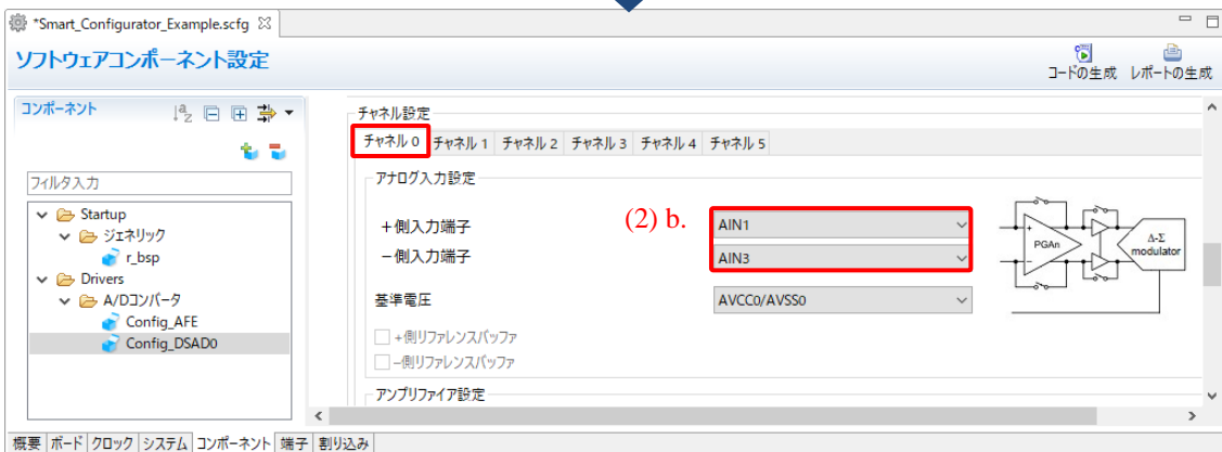
図 4-36 Config_DSAD0 の設定
