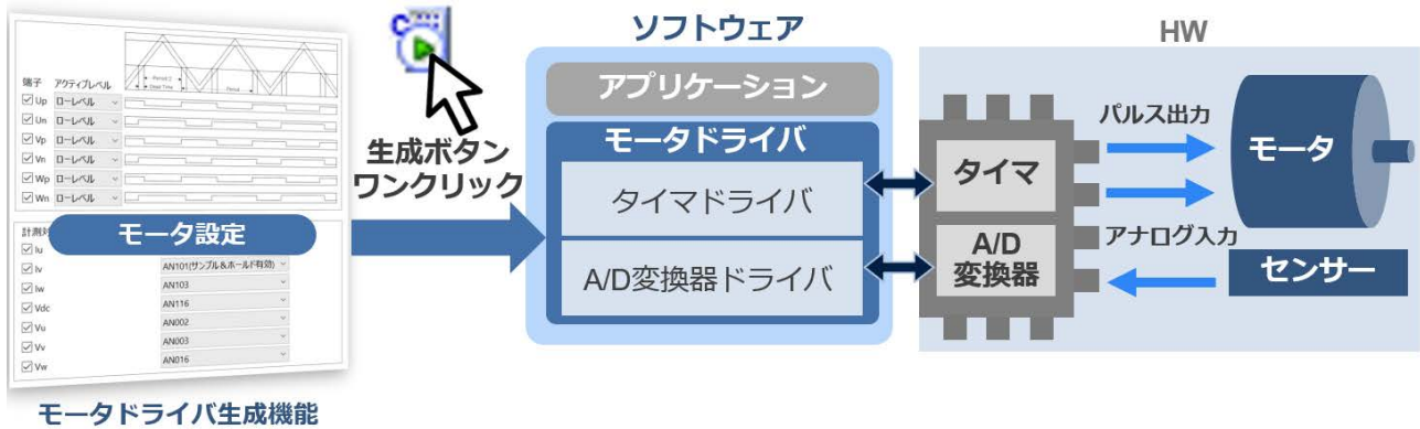
図 4-39 モータドライバジェネレータ
