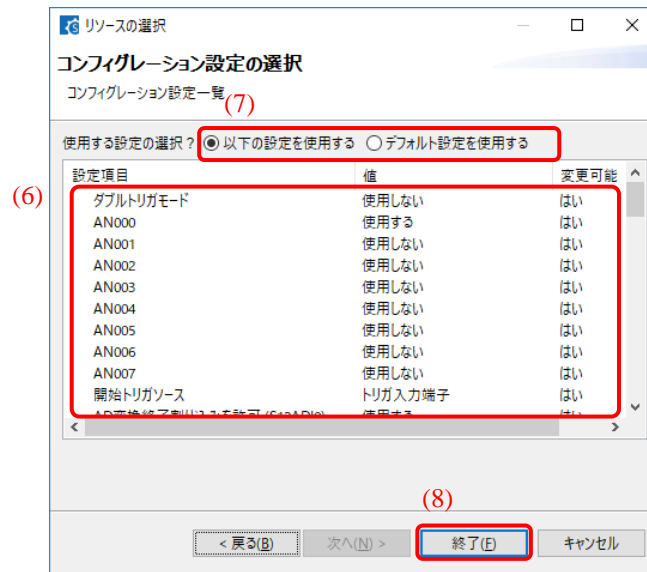
図 4-18 新しいリソース設定の確認
