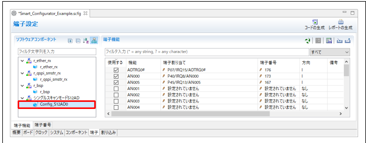
図 6-5 Config_S12AD0の端子設定
