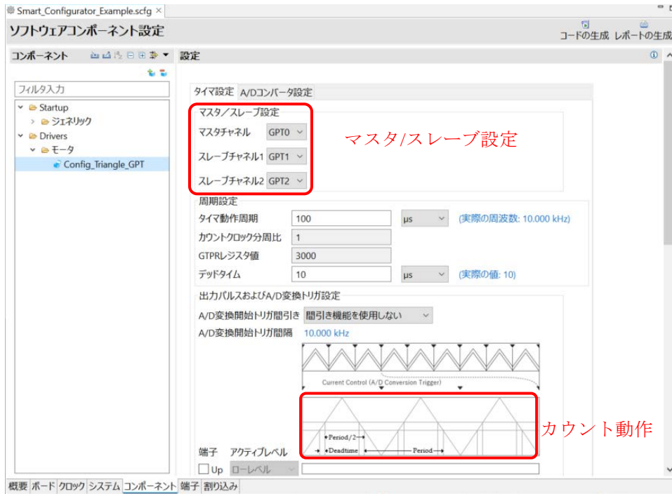
図 4-45 タイマ設定(1)
