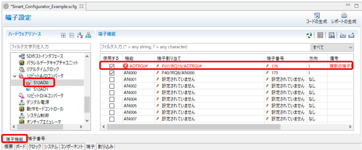
図 5-2 端子の競合
