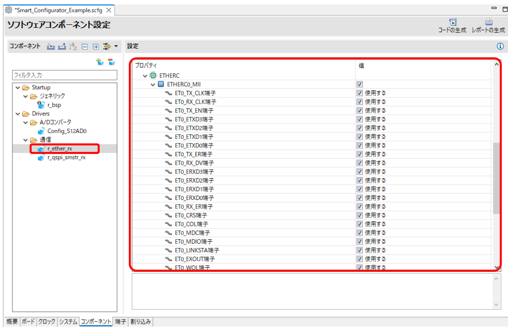
図 4-27 r_ether_rx の端子設定
