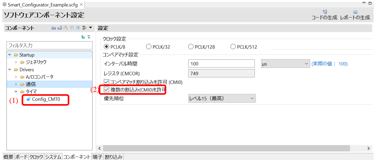
図 4-68 コンポーネントページの多重割り込み設定
