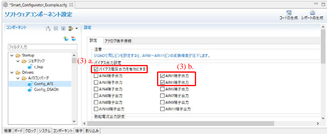
図 4-37 Config_AFE の設定
