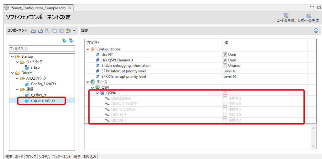
図 4-28 r_qspi_smstr_rx の端子設定
