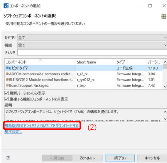
図 4-21 他のソフトウェアコンポーネントのダウンロード
