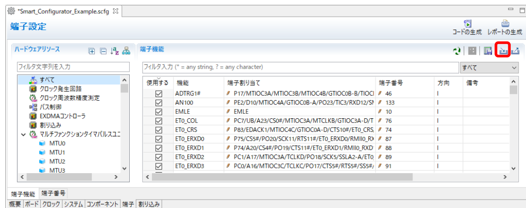
図 4-56 端子設定を XML ファイルからインポートする
