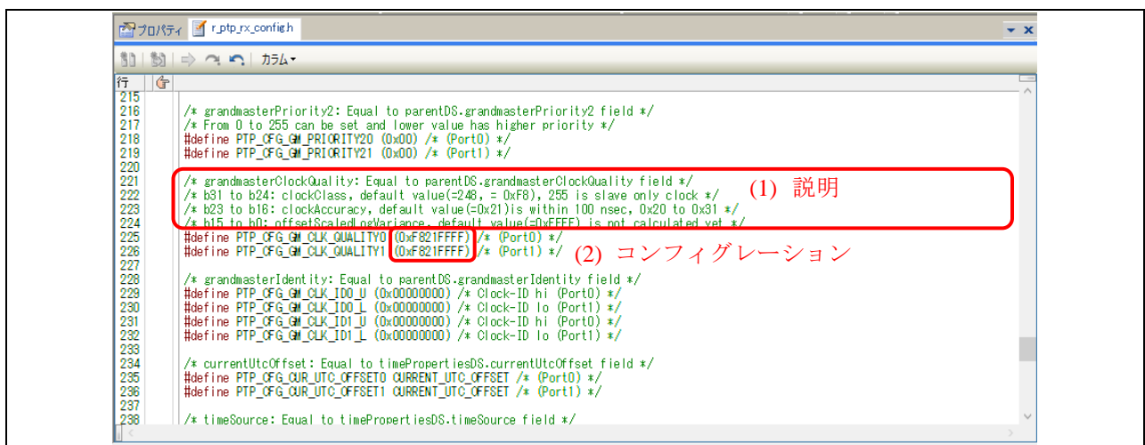
図 6-10 r_XXX_config.h ( r_ether_rx_config.h ) の例
