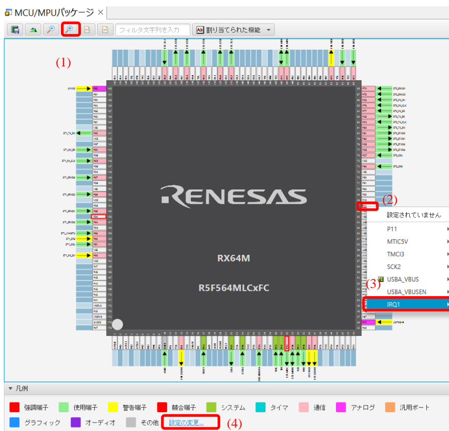
図 4-53 MCU/MPU パッケージを使用した端子設定
