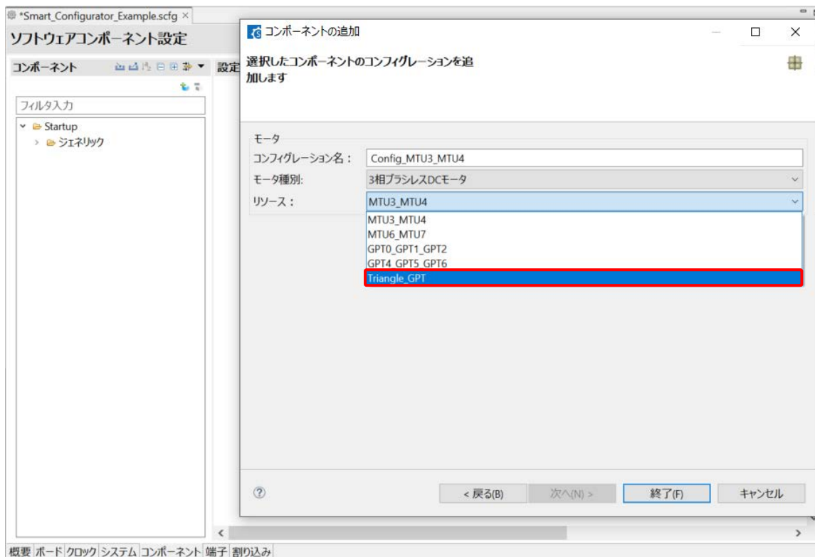
図 4-44 モータリソースの選択
