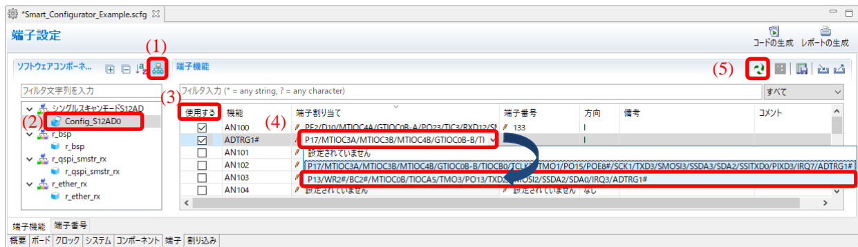
図 4-52 端子設定- [端子機能] リストの端子配置設定
