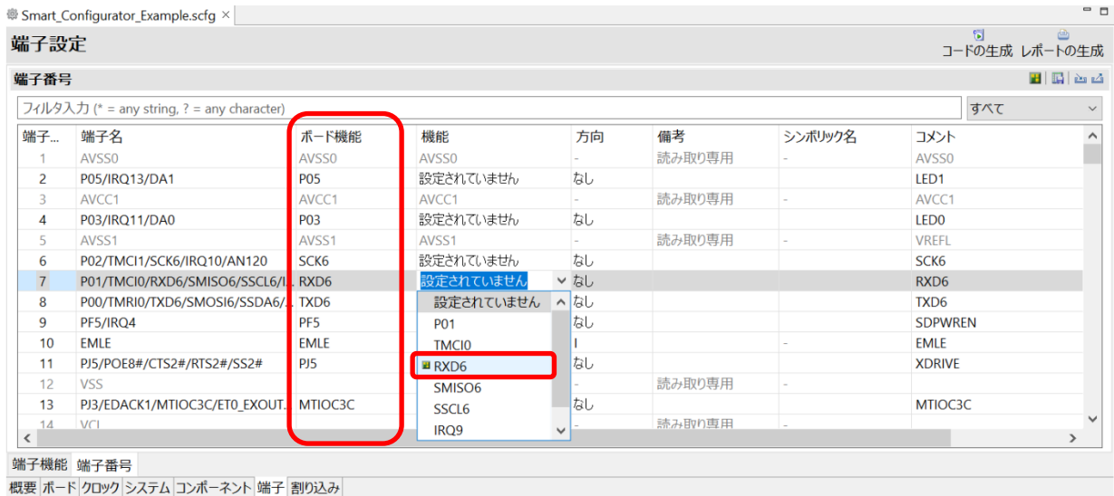
図 4-51 端子ページ（端子番号）
