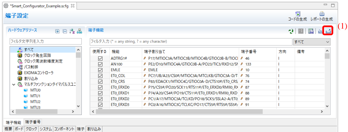
図 4-55 端子設定を XML ファイルへエクスポートする
