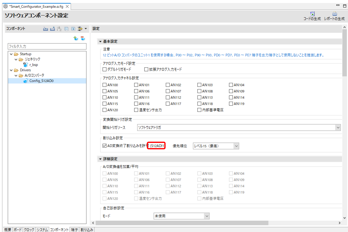
図 4-19 自動的に更新されるリソース
