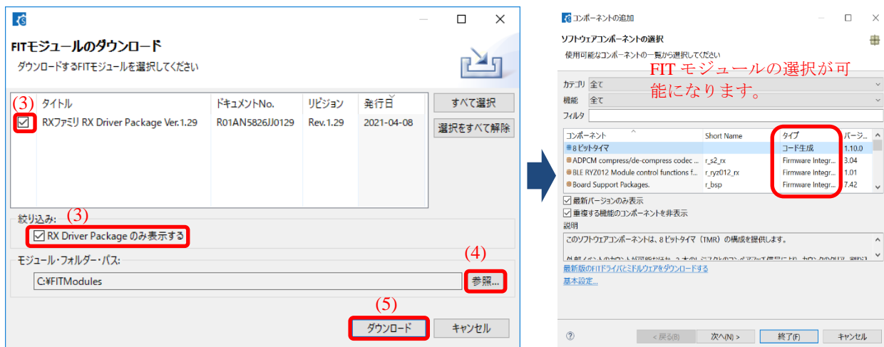
図 4-25 FIT モジュールのダウンロード
