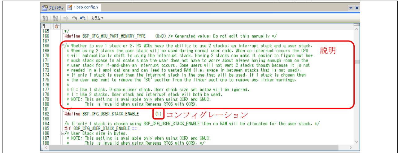
図 6-9 r_bsp_config.h
