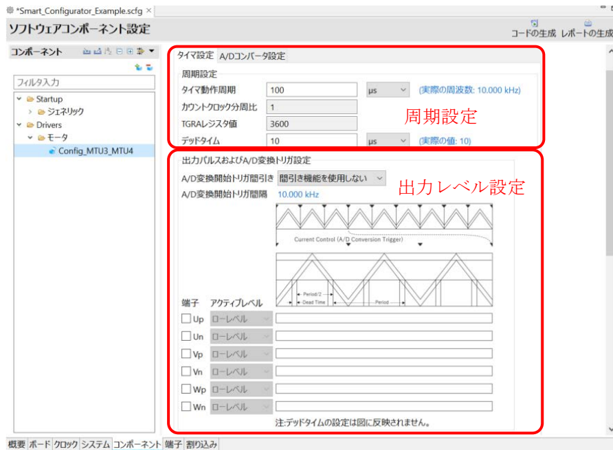
図 4-41 タイマ設定(1)
