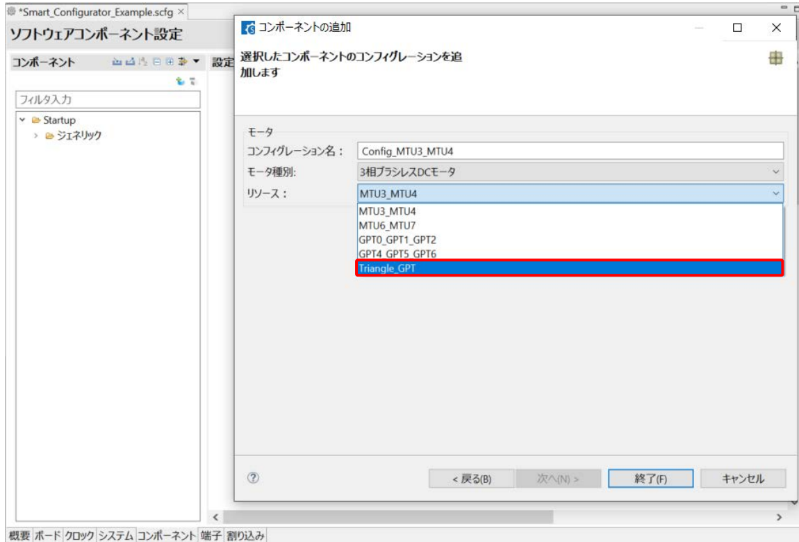
図 4-44 モーターリソースの選択
