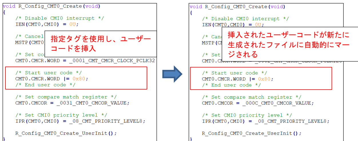
図 10-2 ユーザーコードの保護機能
