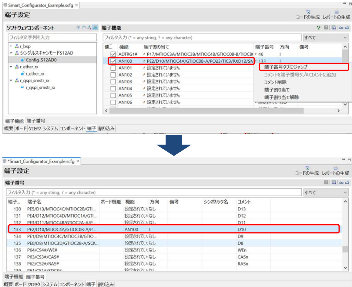
図 4-54 端子機能から端子番号への移動
