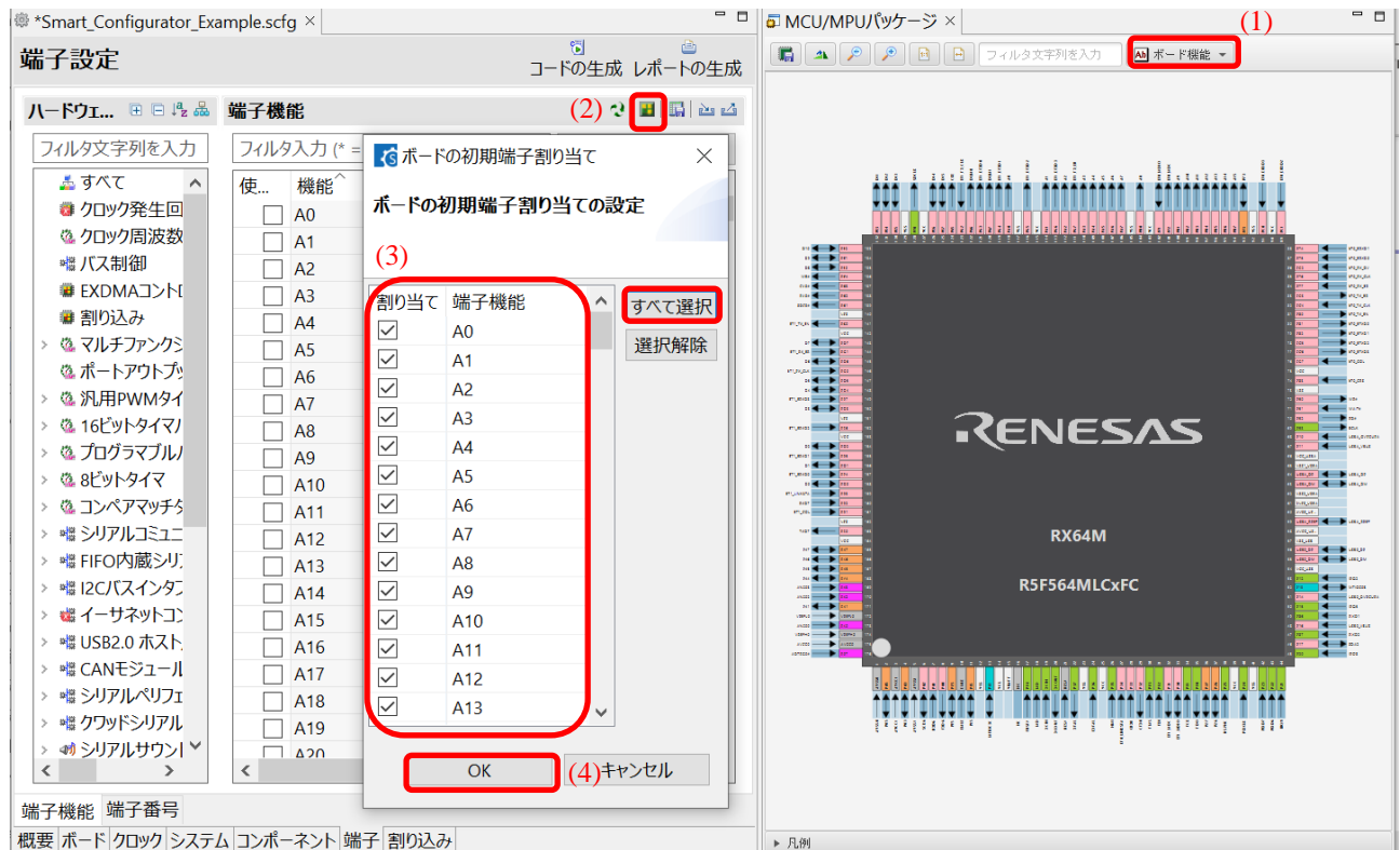
図 4-57 ボードの初期端子設定
