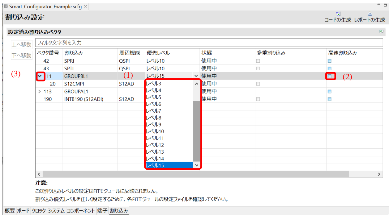
図 4-66 割り込み設定
