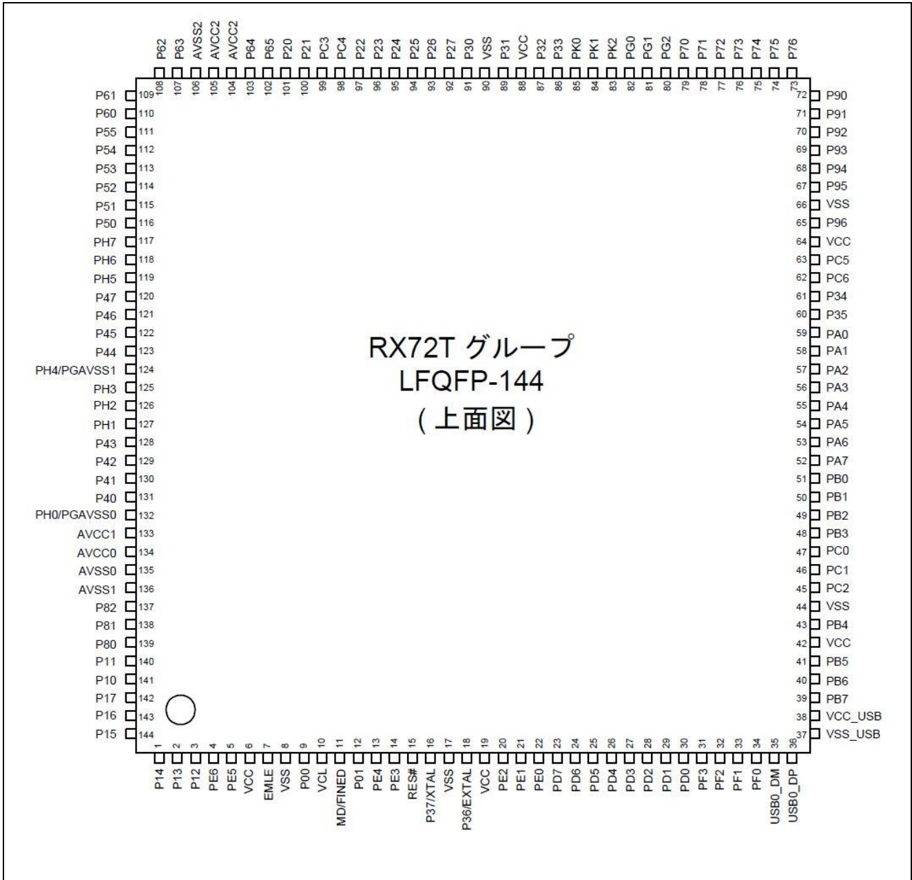
図 6.1 RX72T ピン配置
