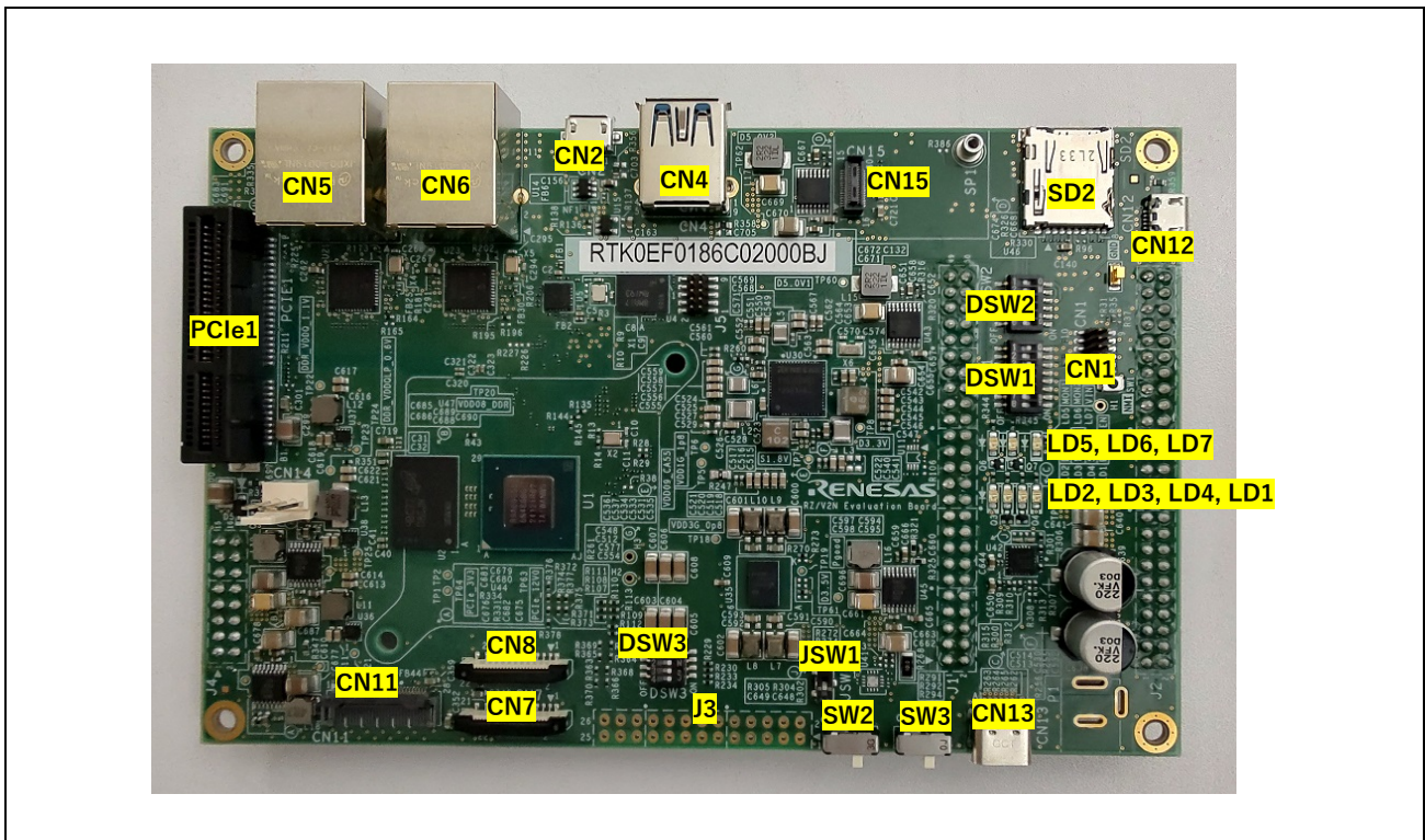
図 3.1-1 RZ/V2N Evaluation Board 部品配置図 (部品面)
