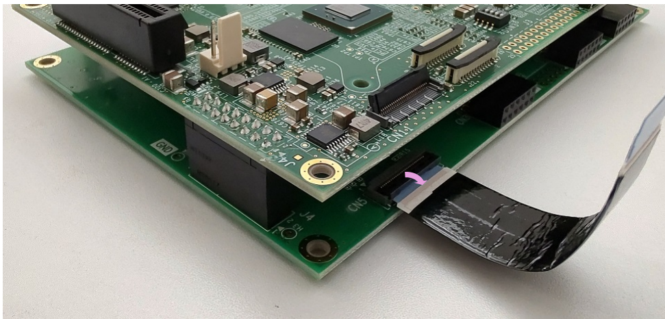
図 2.1-1 FFC を RZ/V2H EVK Expansion Board に接続
