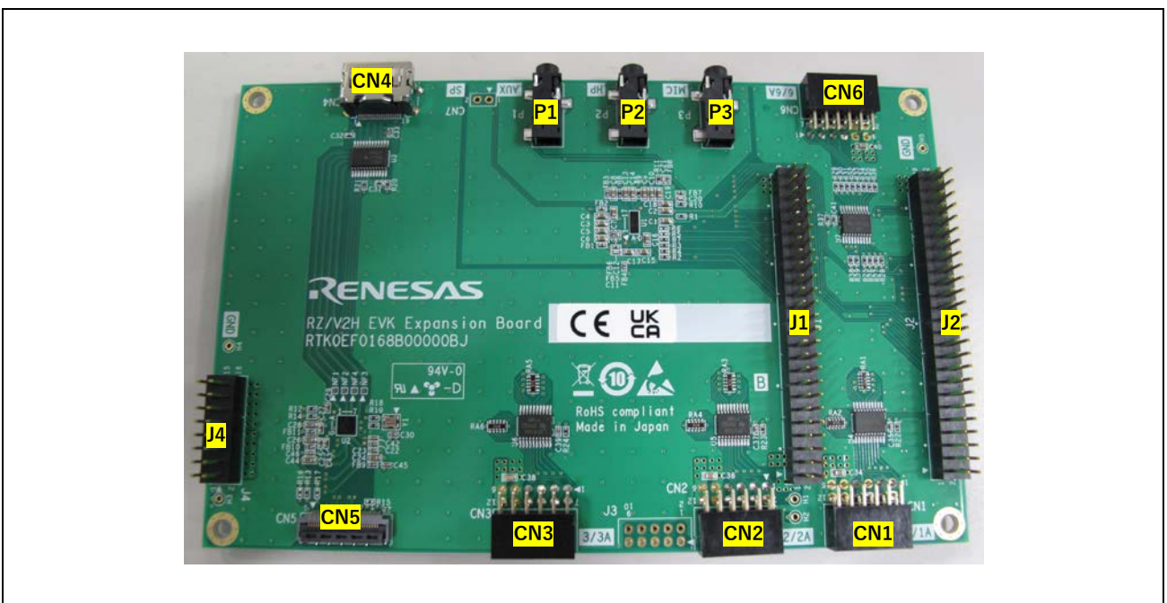
図 3.1-3 RZ/V2H EVK Expansion Board 部品配置図 (部品面)
