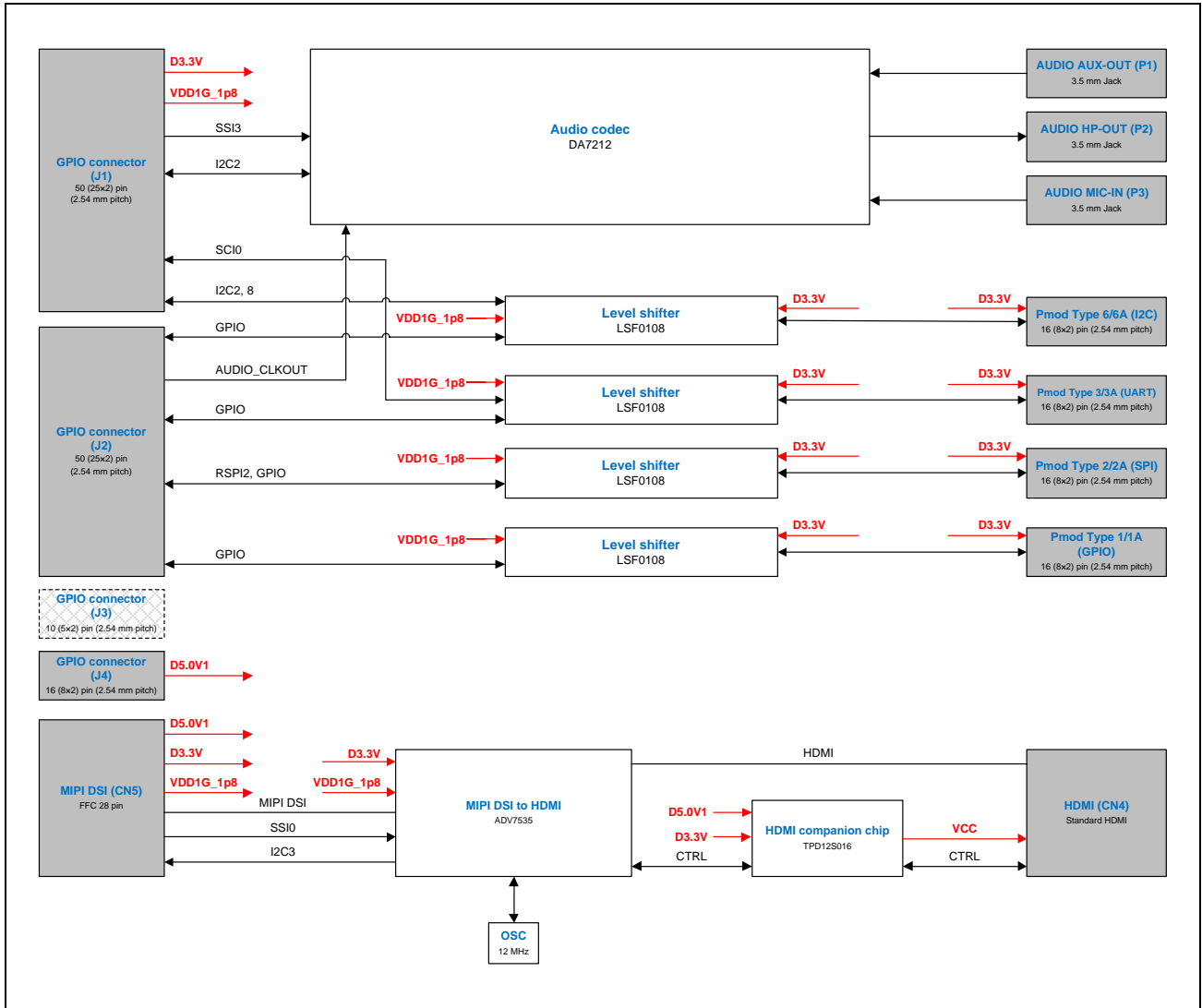
図 1.2-2 RZ/V2H EVK Expansion Board ブロック図
