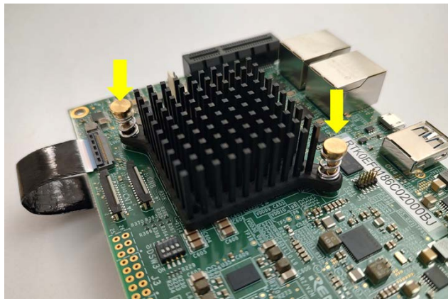
図 5.2-1 ヒートシンクを RZ/V2N Evaluation Board に接続
