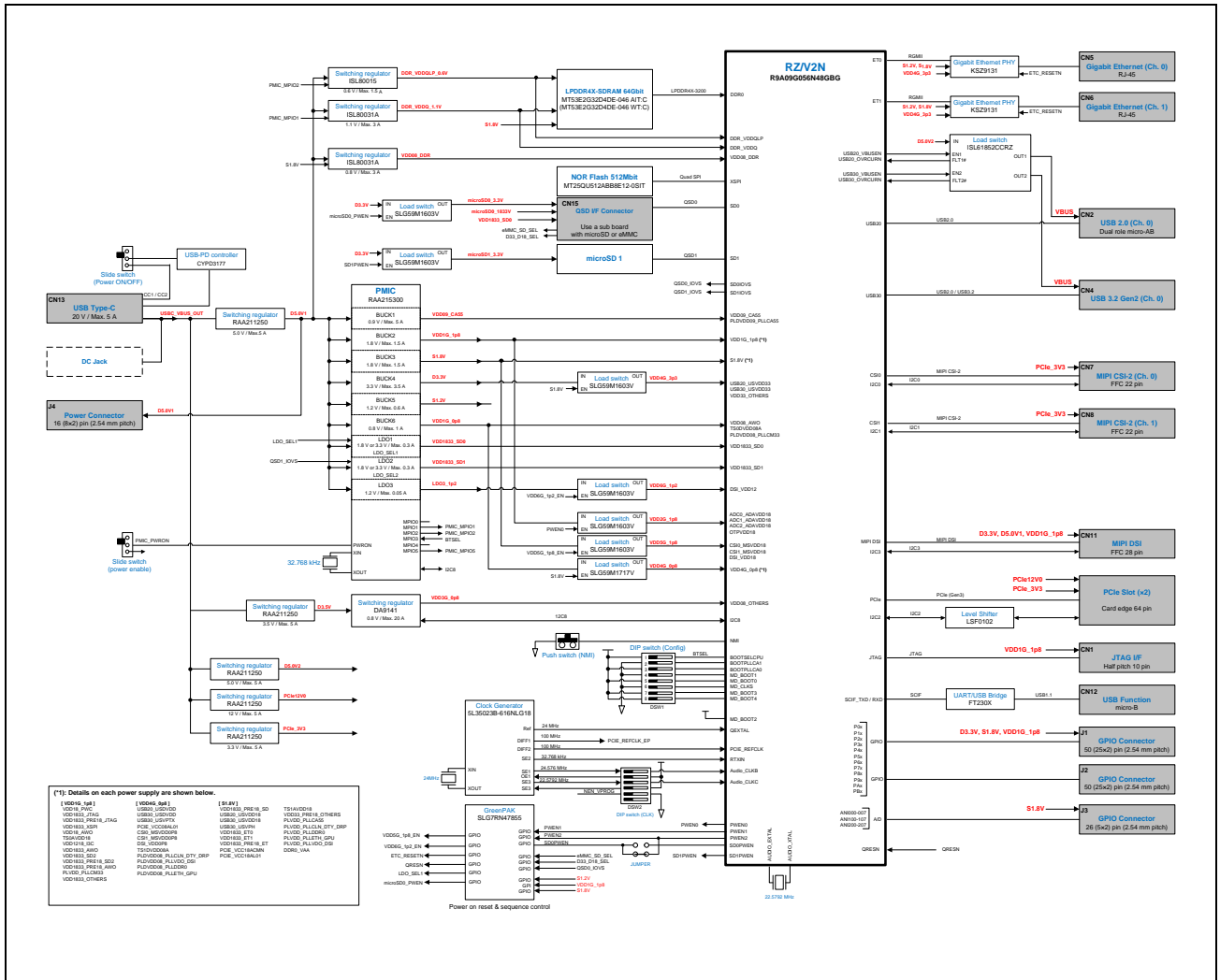
図 1.2-1 RZ/V2N Evaluation Board ブロック図
