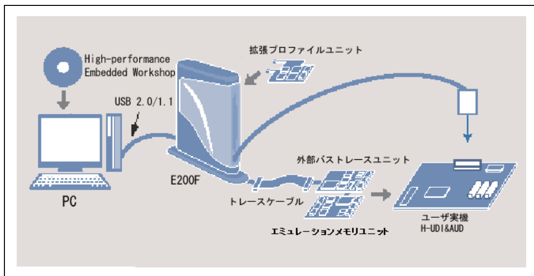
図 1.1 E200F エミュレータを使用したシステム構成外観
