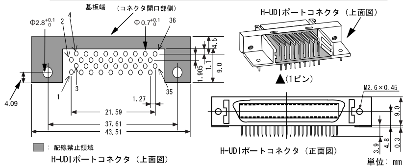
図 2.1 H-UDI ポートコネクタのピン配置(36 ピン)
