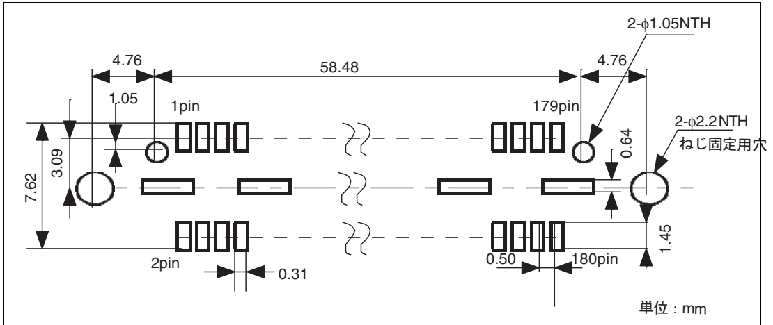
図 2.4 推奨フットパターン（コネクタ実装面図）
