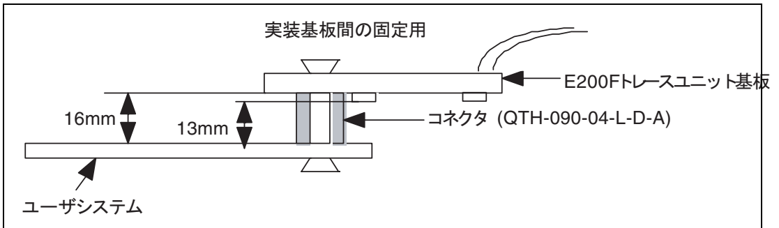
図 2.5 部品の高さ制限
